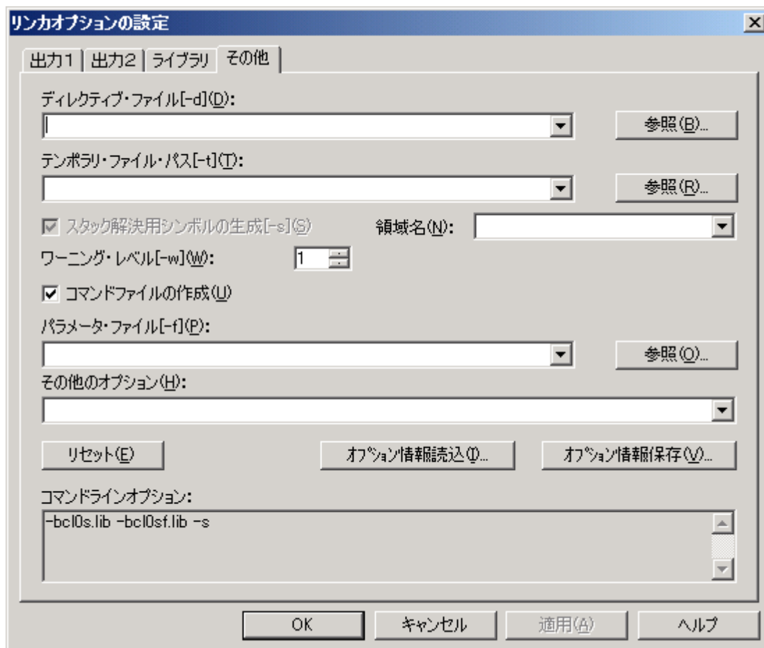
図 3-23 〈リンカオプションの設定〉ダイアログ
