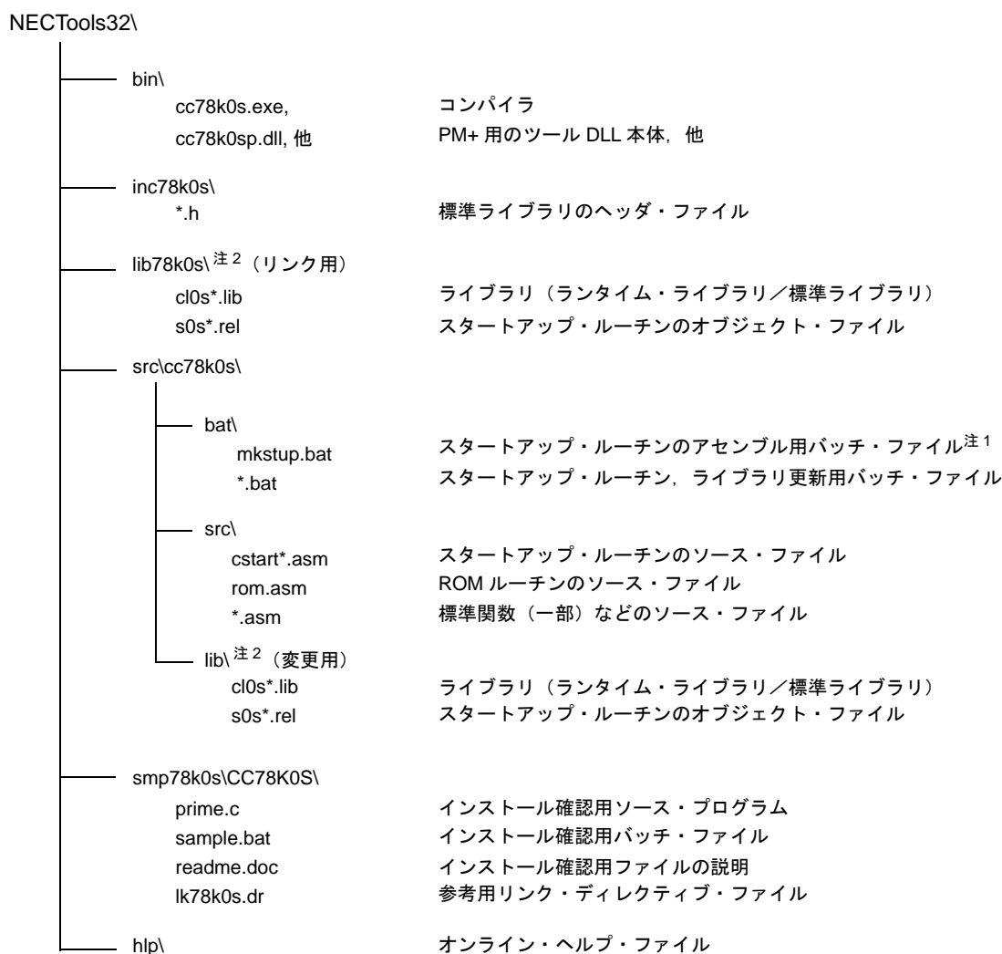
図 2-1 フォルダ構成
