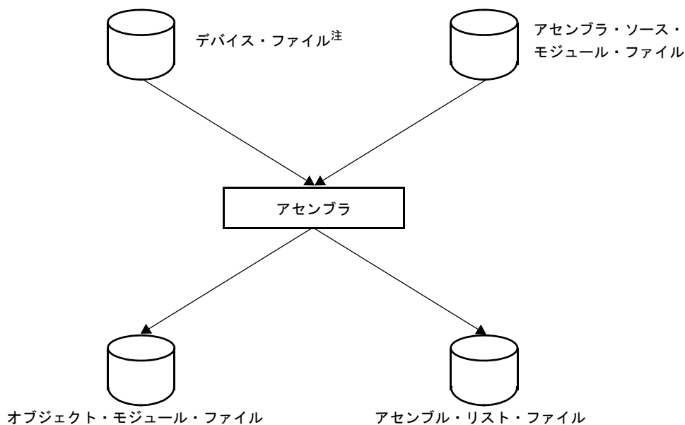
図 1-6 アセンブラの機能
