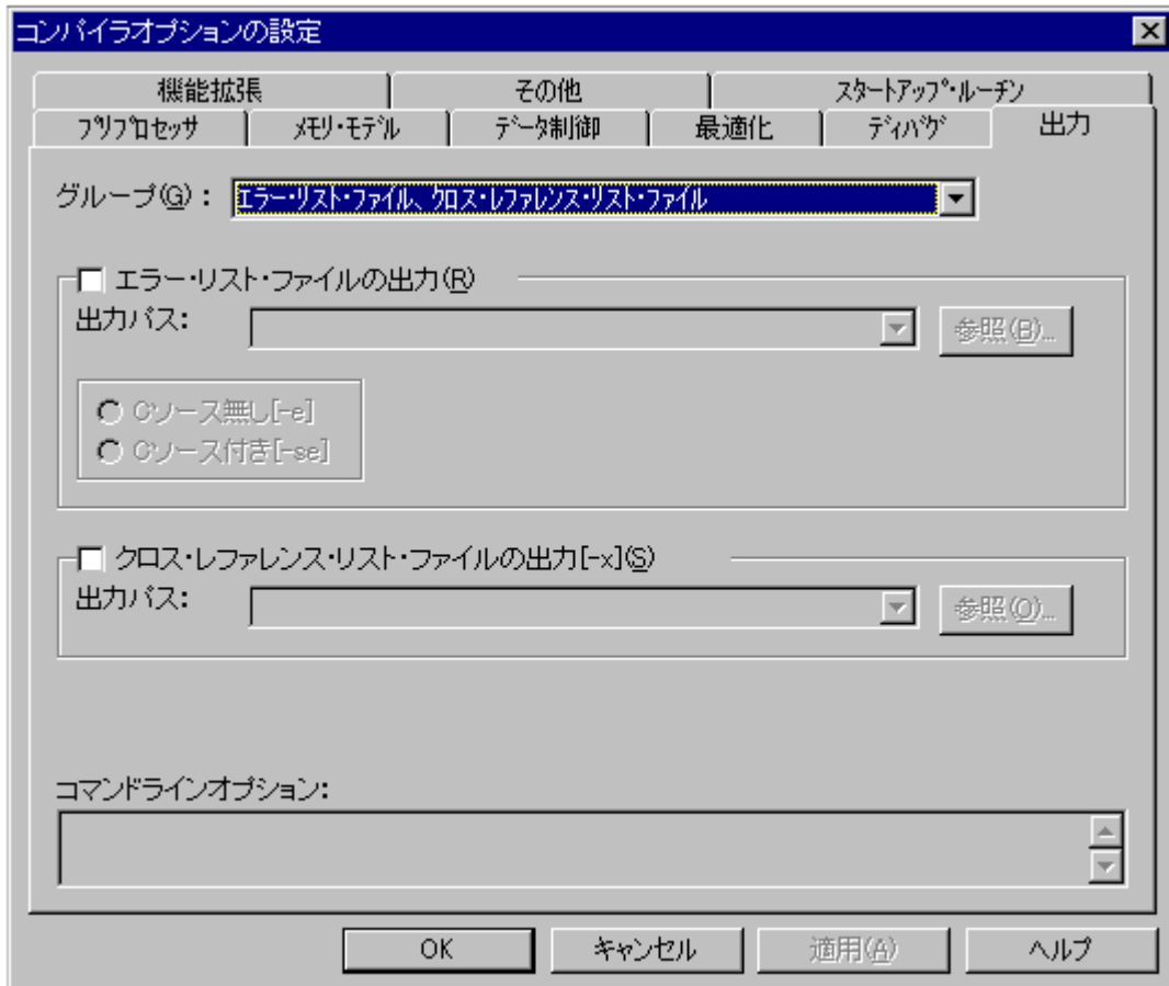
図 3-17 <コンパイラオプションの設定> ダイアログ (“エラー・リスト・ファイル、クロス・レファレンス・リスト・ファイル” 選択時)
