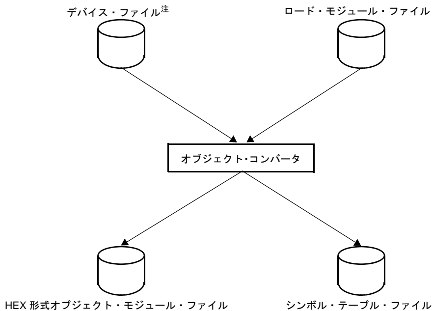
図 1-8 オブジェクト・コンバータの機能
