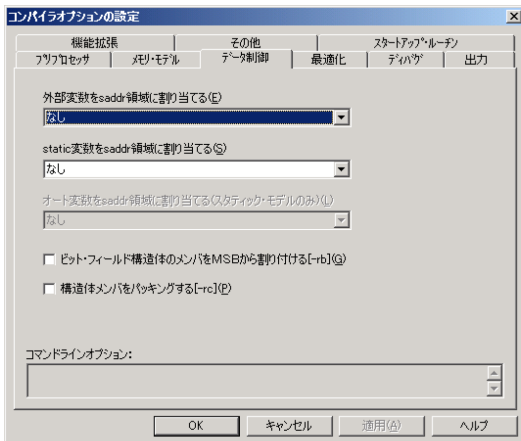
図 3-9 &lt;コンパイラオプションの設定&gt; ダイアログ ([データ制御] タブ選択時)
