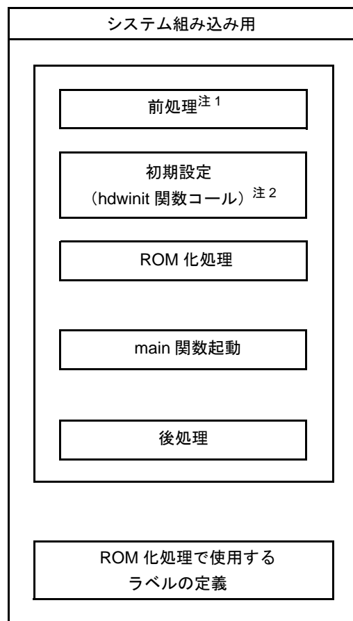
図8-1 スタートアップ・ルーチンの概要
