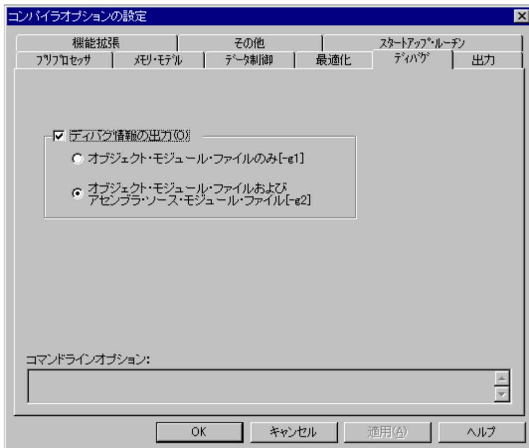
図 3-14 &lt;コンパイラオプションの設定&gt; ダイアログ ([ディバグ] タブ選択時)
