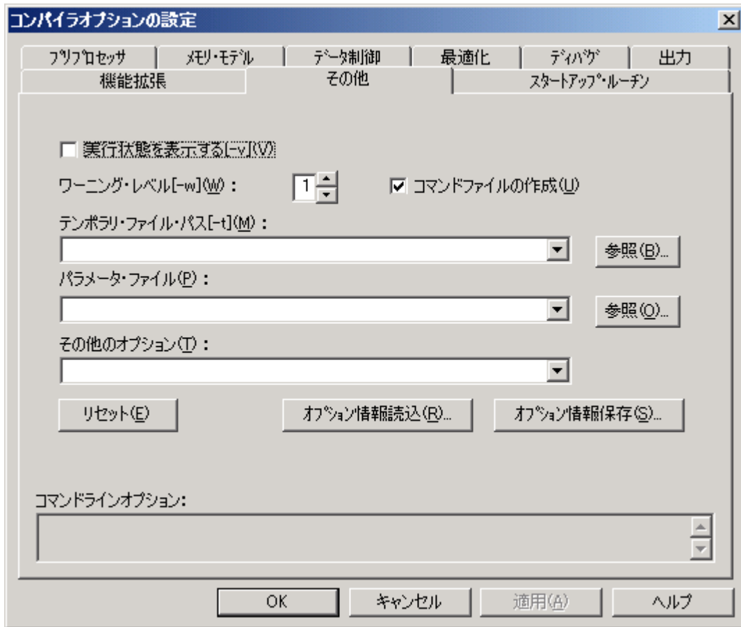
図 3-20 &lt;コンパイラオプションの設定&gt; ダイアログ ([その他] タブ選択時)
