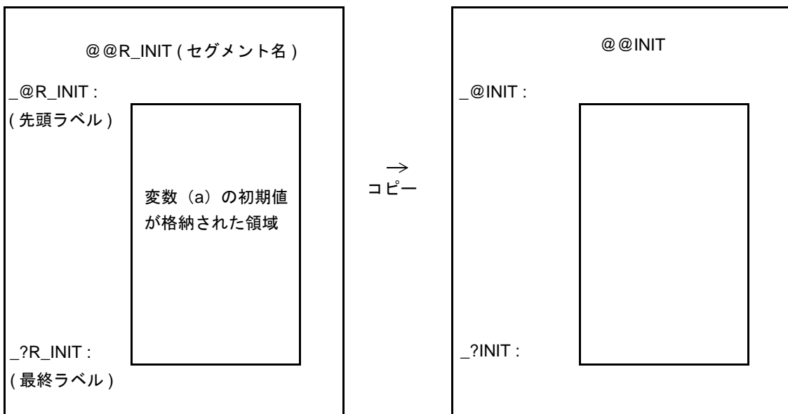
図 8-2 ROM 化処理
