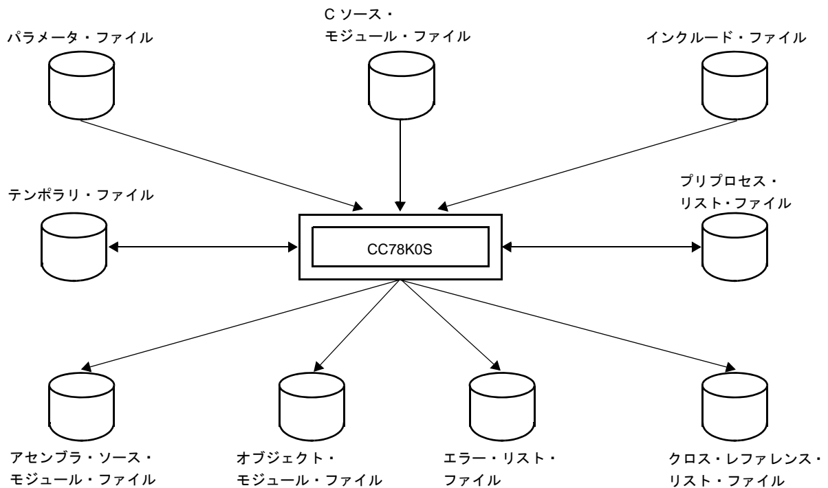
図 3-24 C コンパイラの入出力ファイル
