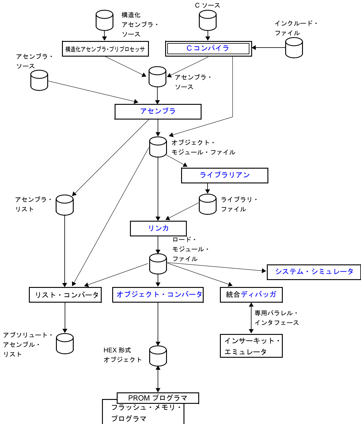
図 1-3 CC78K0S によるプログラム開発手順
