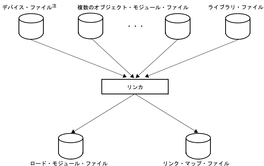
図 1-7 リンカの機能
