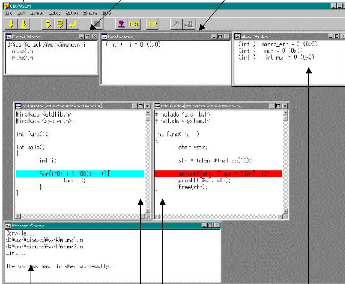
図1：CB79SIMのウィンドウ構成図
