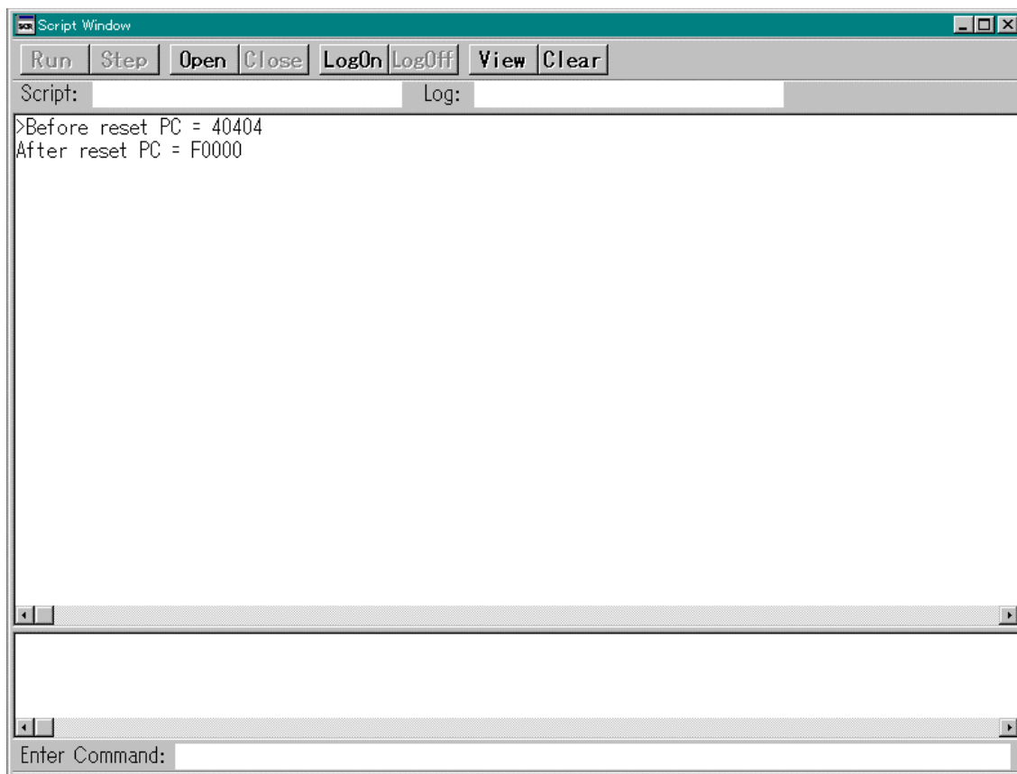
図 1 4： カスタムコマンドプログラム m_reset.p の実行例
