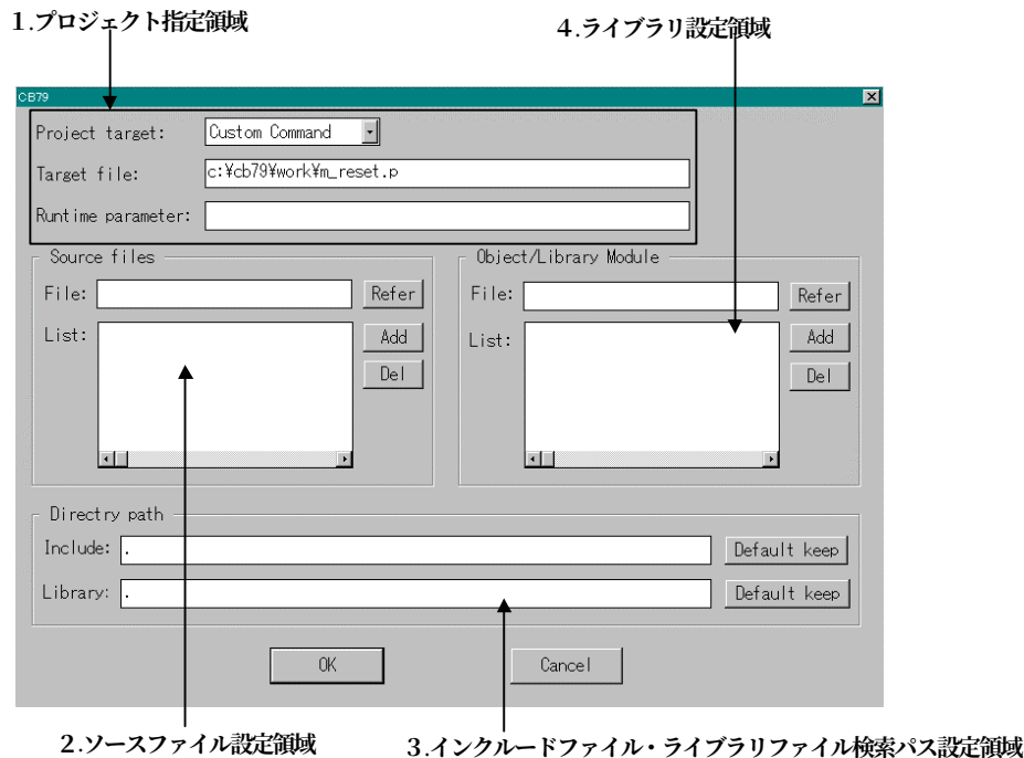
図 2 2：セットアップダイアログの構成図
