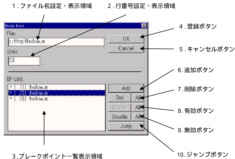
図 2 7 : ブレークポイントダイアログの構成図
