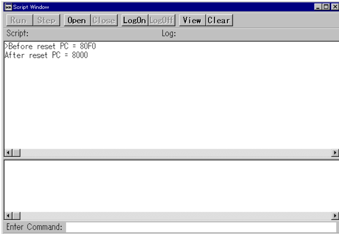
図 1 4 : カスタムコマンドプログラム m_reset.p の実行例
