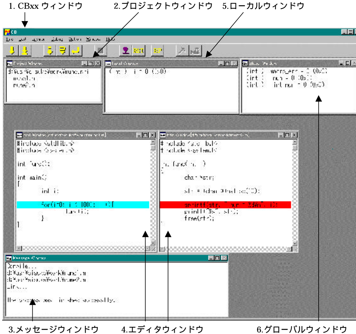
図1：CB38SIMのウィンドウ構成図
