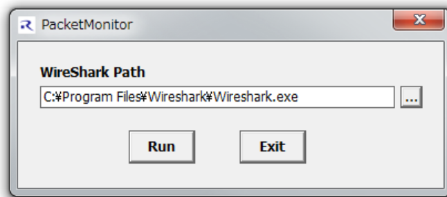
図 12-2 Wireshark.exe の選択
