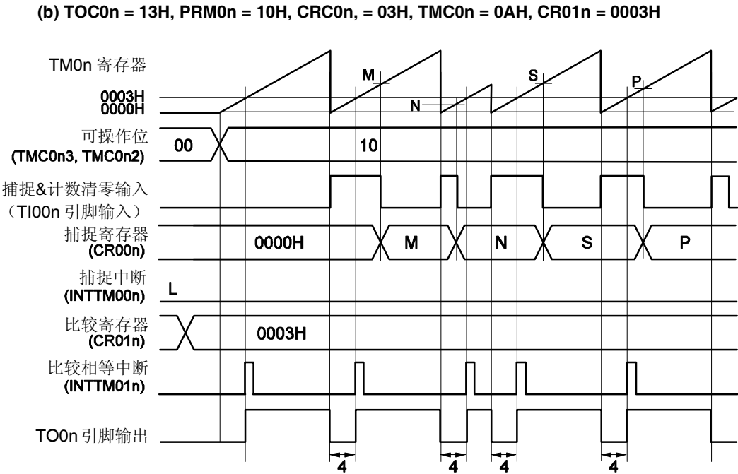
图 7-32 清零&启动模式(通过 TI00n 引脚有效沿输入进入) 时序示例 (CR00n: 捕捉寄存器, CR01n: 比较寄存器) (2/2)
