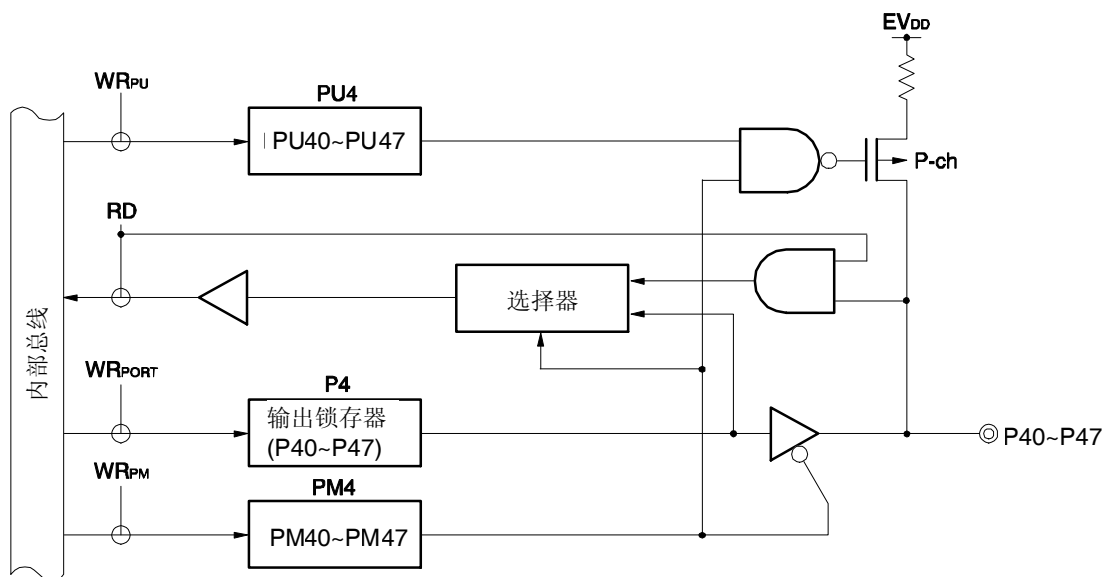
图 5-15. 的框图 P40 ~ P47
