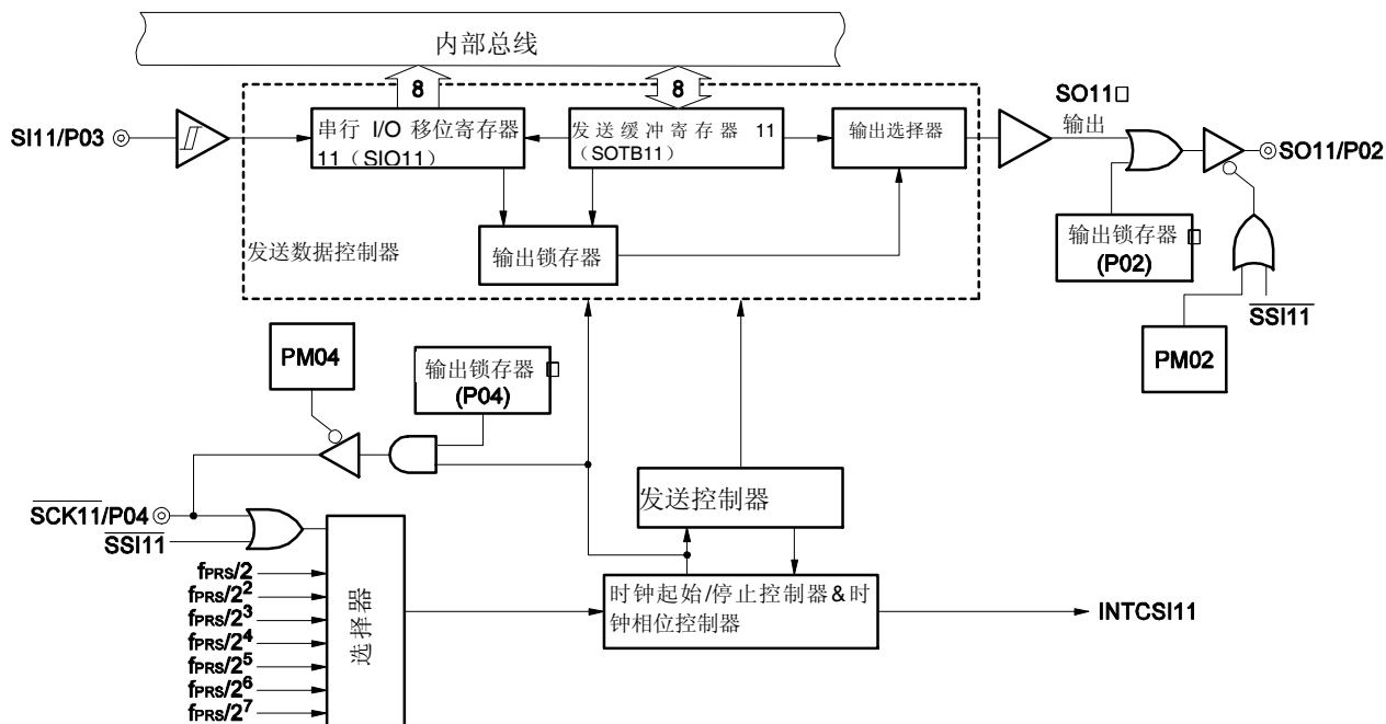
图 16-2 串行接口 CSI11 的框图
