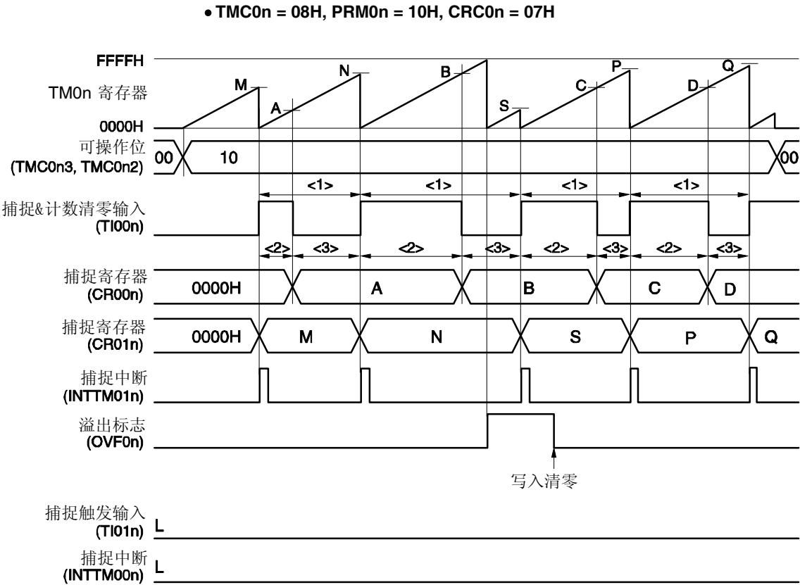
图 7-55. 脉冲宽度测量时序示例(3)
