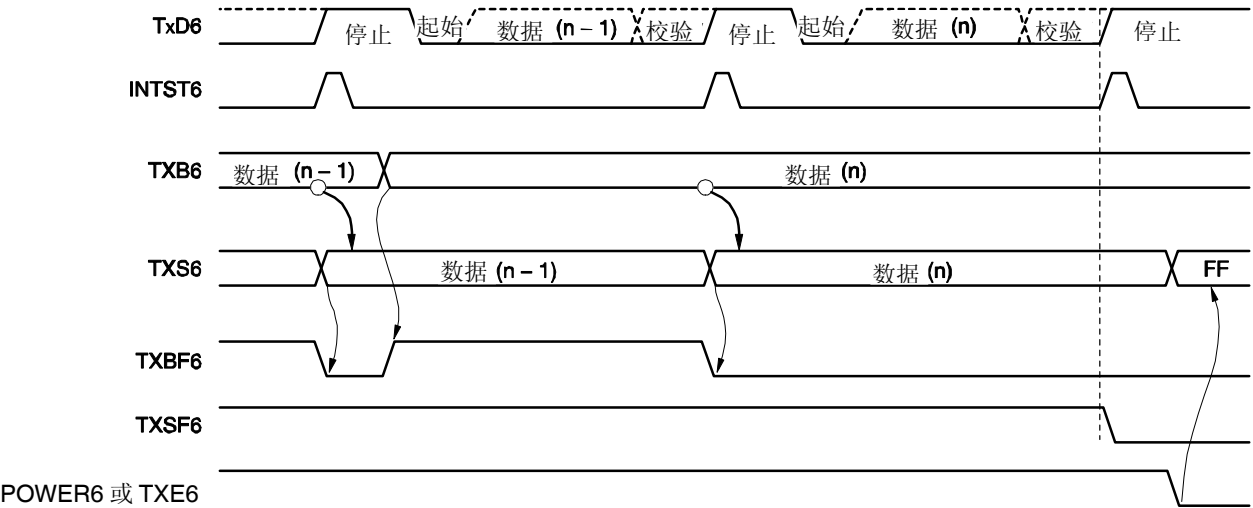
图 15-18 结束连续发送的时序
