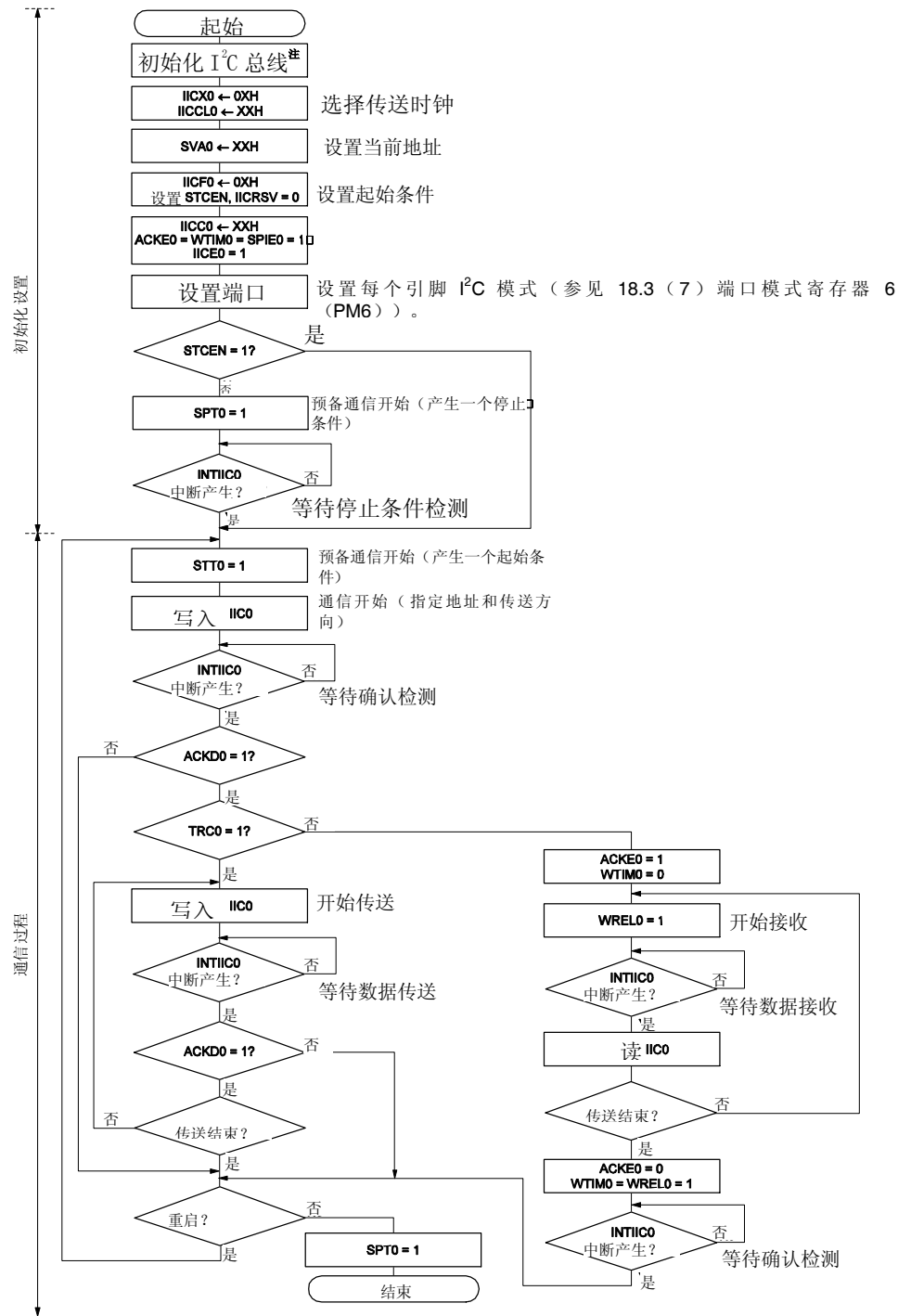
图 18-23. 主设备操作(单主设备系统)
