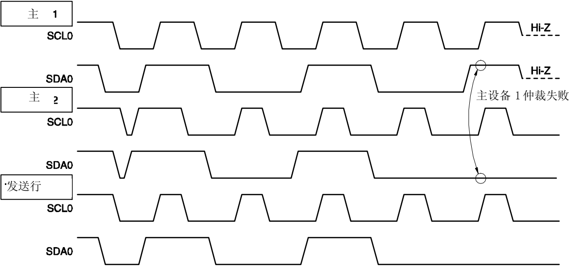
图 18-19. 仲裁时序举例
