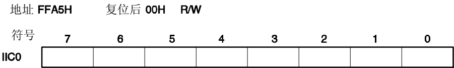
图 18-3. IIC 移位寄存器 0 的格式 (IIC0)
