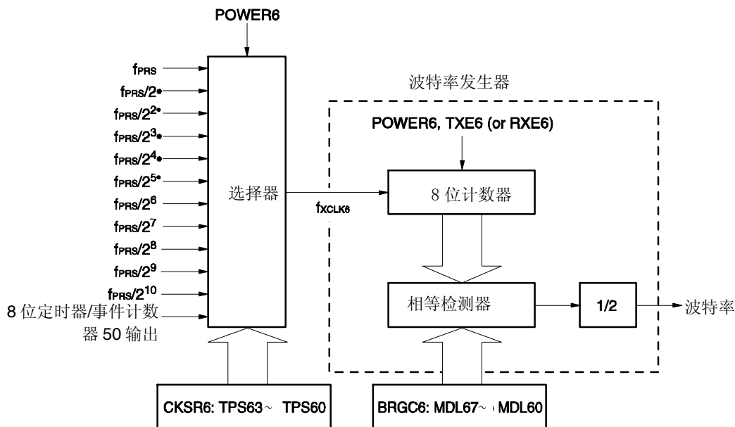
图 15-24 波特率发生器的配置
