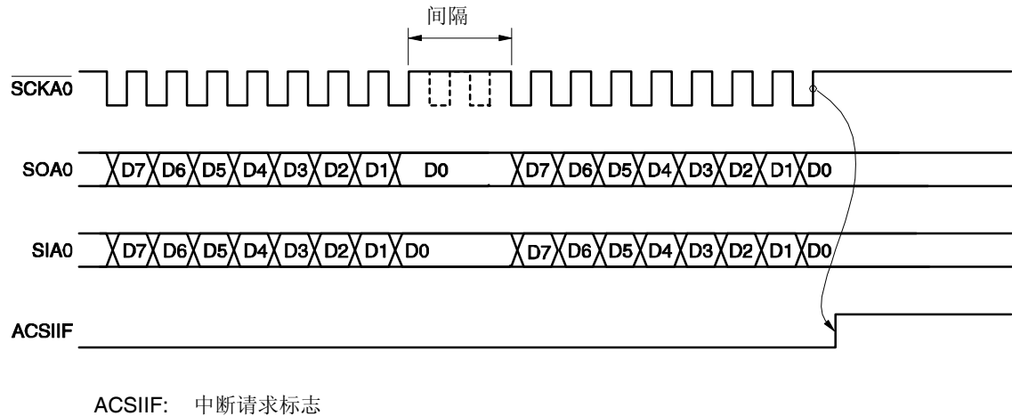
图 17-28 自动发送/接收间隔时间举例 (当 ADTI0 = 00H, STBE0 = 1, BUSYE0 = 0 (两个时钟))
