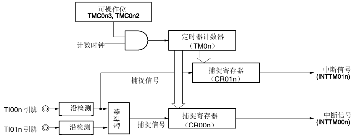
图 7-41 自由运行定时器模式的框图 (CR00n: 捕捉寄存器, CR01n: 捕捉寄存器)
