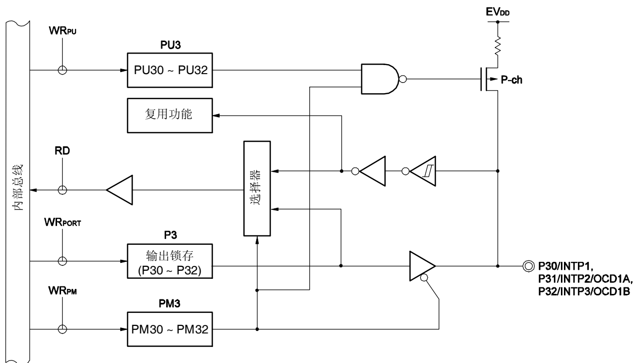
图 5-13. P30 ~ P32 的框图
