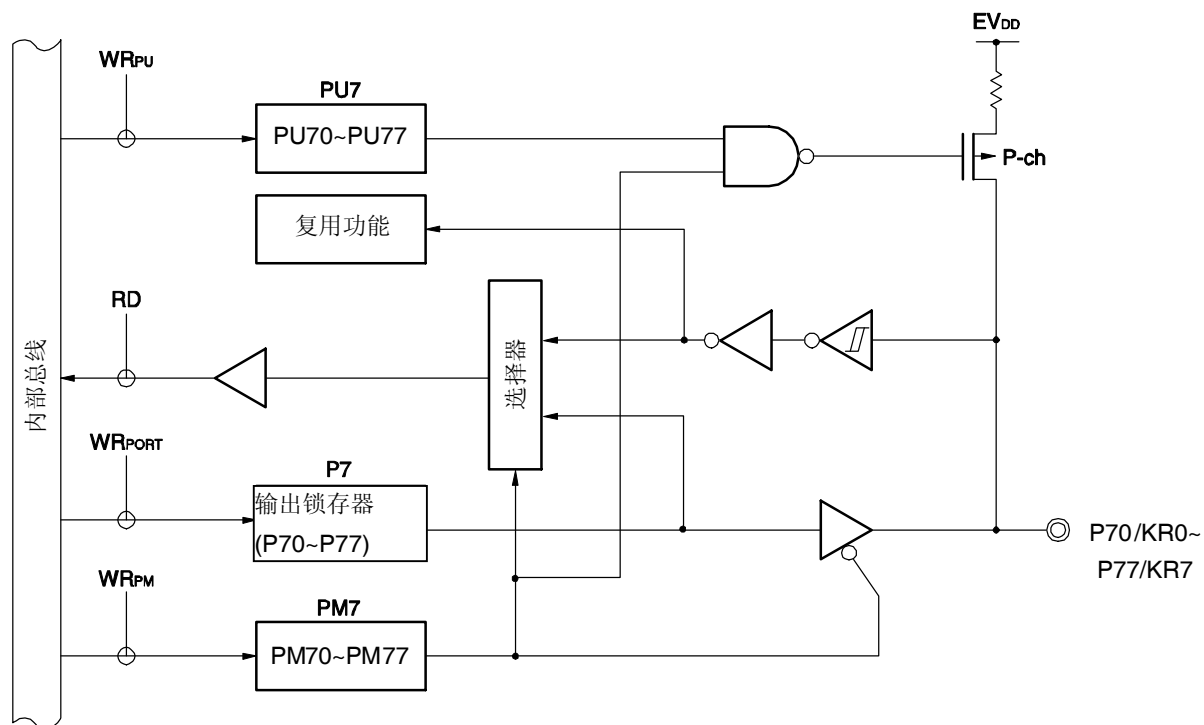
图 5-21. P70~P77 的框图
