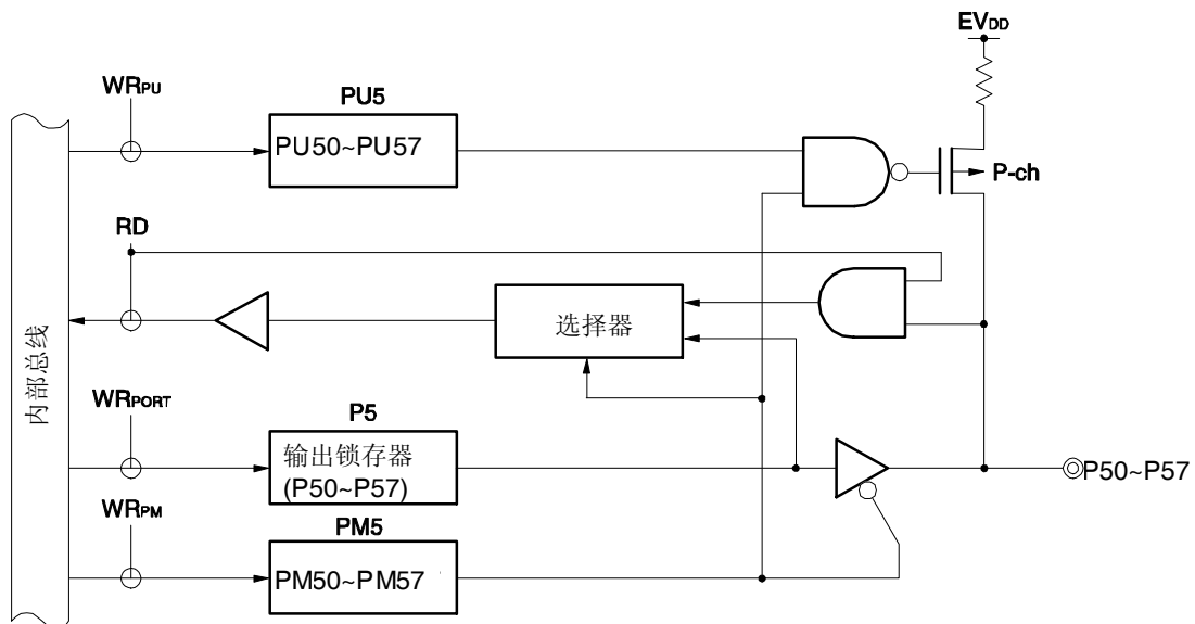
图 5-16. P50~P57 的框图
