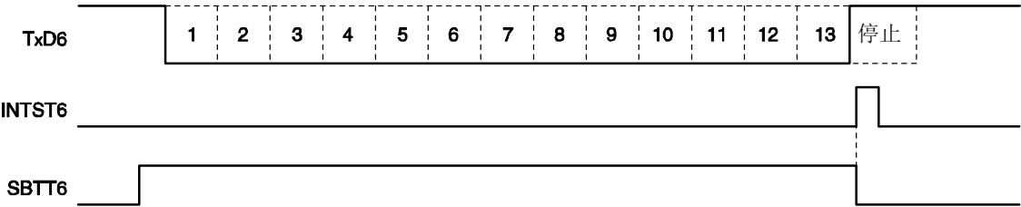
图 15-22. SBF 发送
