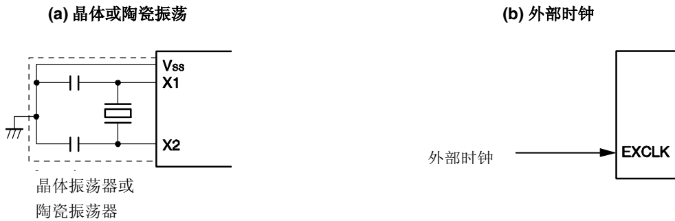
图 6-12. X1 振荡器的外部电路示例
