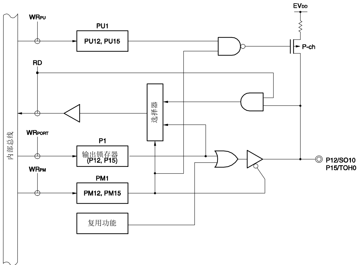
图 5-9. P12 和 P15 的框图
