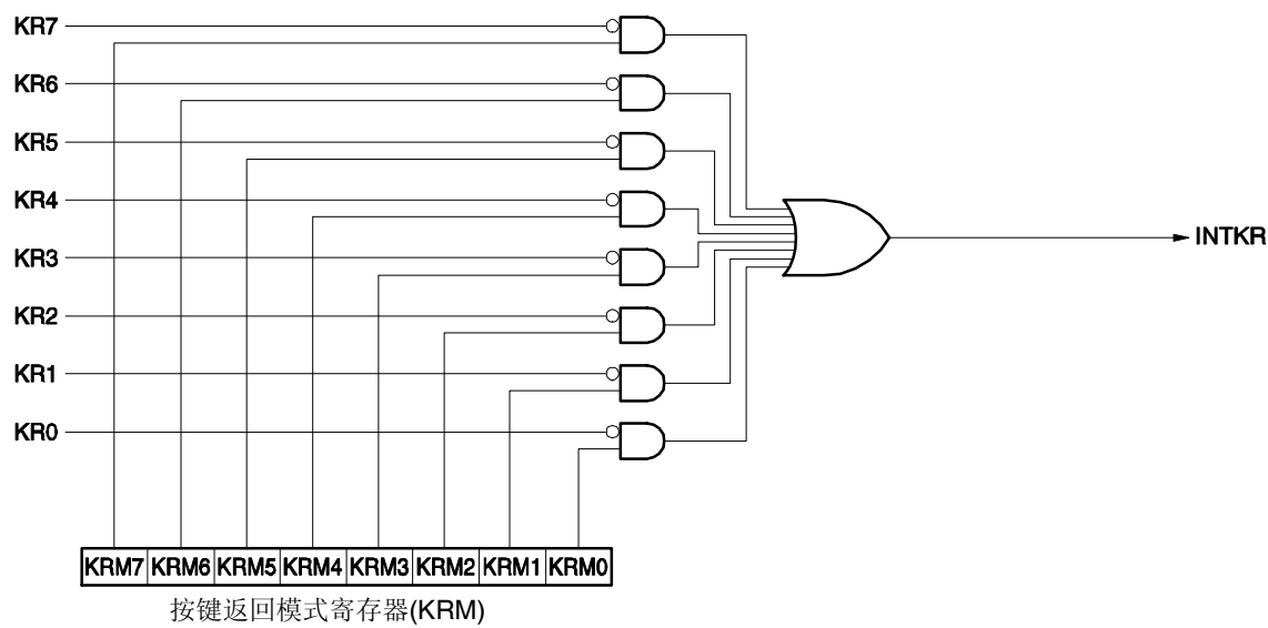
图 21-1. 按键中断框图
