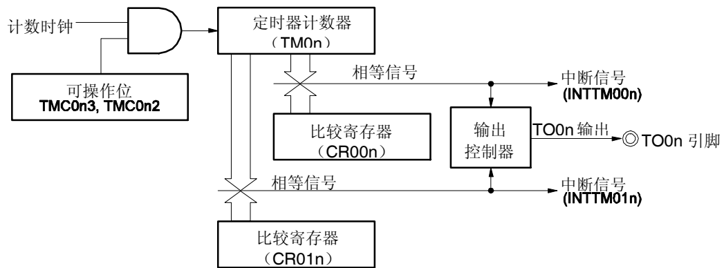
图 7-37 自由运行定时器模式的框图 (CR00n: 比较寄存器, CR01n: 比较寄存器)
