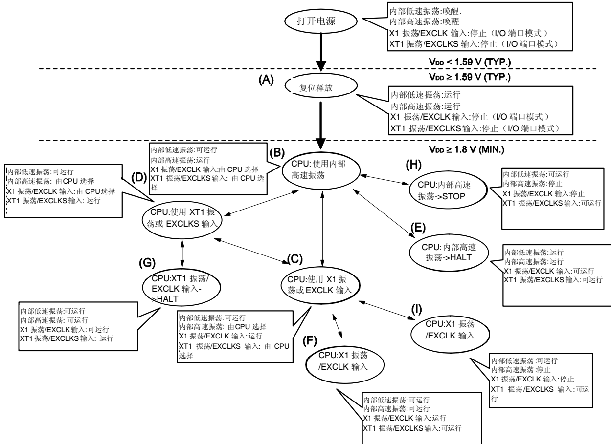
图 6-18. CPU 时钟状态转移图 (设置 1.59 V POC 模式 (选项字节: POCMODE = 0), 78K0/KC2, 78K0/KD2, 78K0/KE2 和 78K0/KF2)
