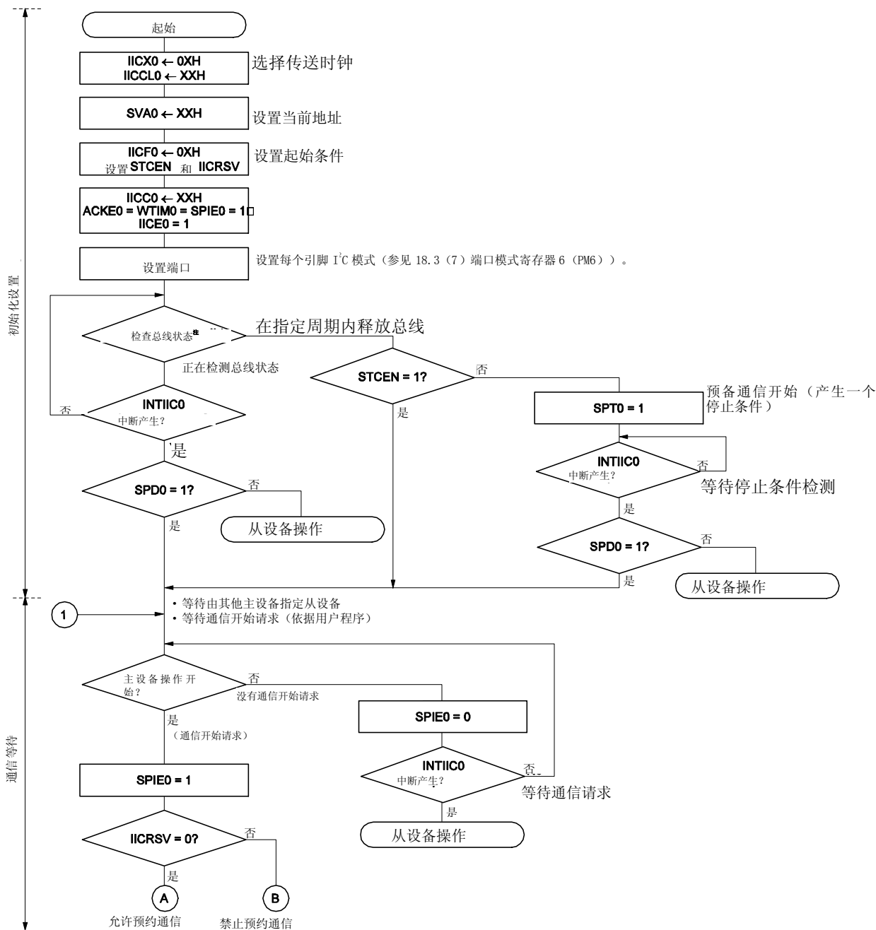
图 18-24. 主设备操作(多主设备系统) (1/3)
