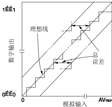
图 13-14. 总误差
