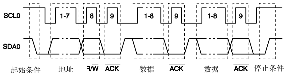
图 18-12. I 2 C 总线串行数据传送时序
