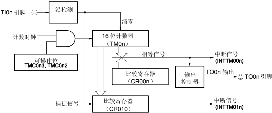
图 7-30 清零&启动模式(通过 TI00n 引脚有效沿输入进入)时序示例 (CR00n: 比较寄存器, CR01n: 捕捉寄存器) (1/2)
