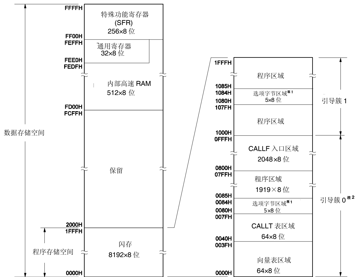
图 3-1. 存储空间映射图 (μPD78F0500A)
