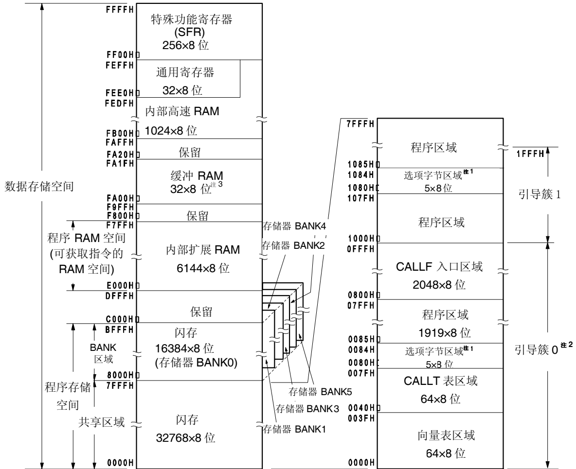
图 3-10. 存储空间映射图 (μPD78F0527A, 78F0537A, 78F0547A)
