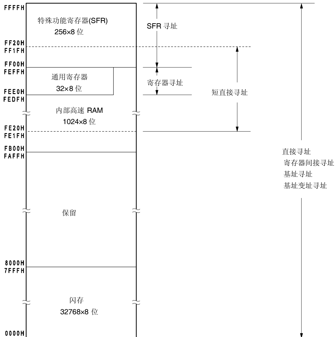
图 3-15. 数据存储空间与寻址方式的对应关系 ( \mu PD78F0503A, 78F0513A, 78F0523A, 78F0533A, 78F0503DA,和 78F0513DA)
