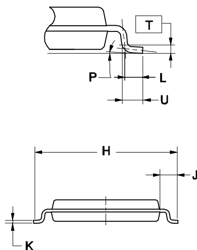
引脚端详图
