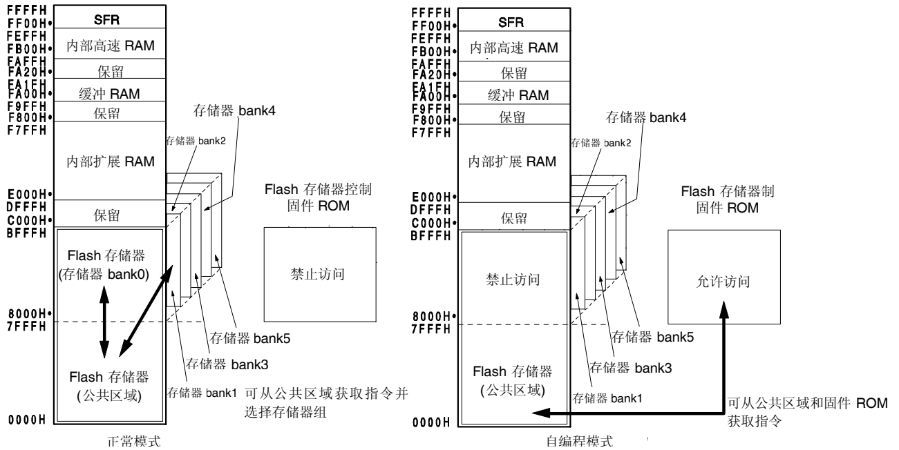
图 27-13. 用于自编程的操作模式和存储器映射(μPD78F0547A)
