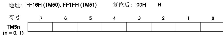
图 8-3. 8 位定时器计数器 5n (TM5n)的格式
