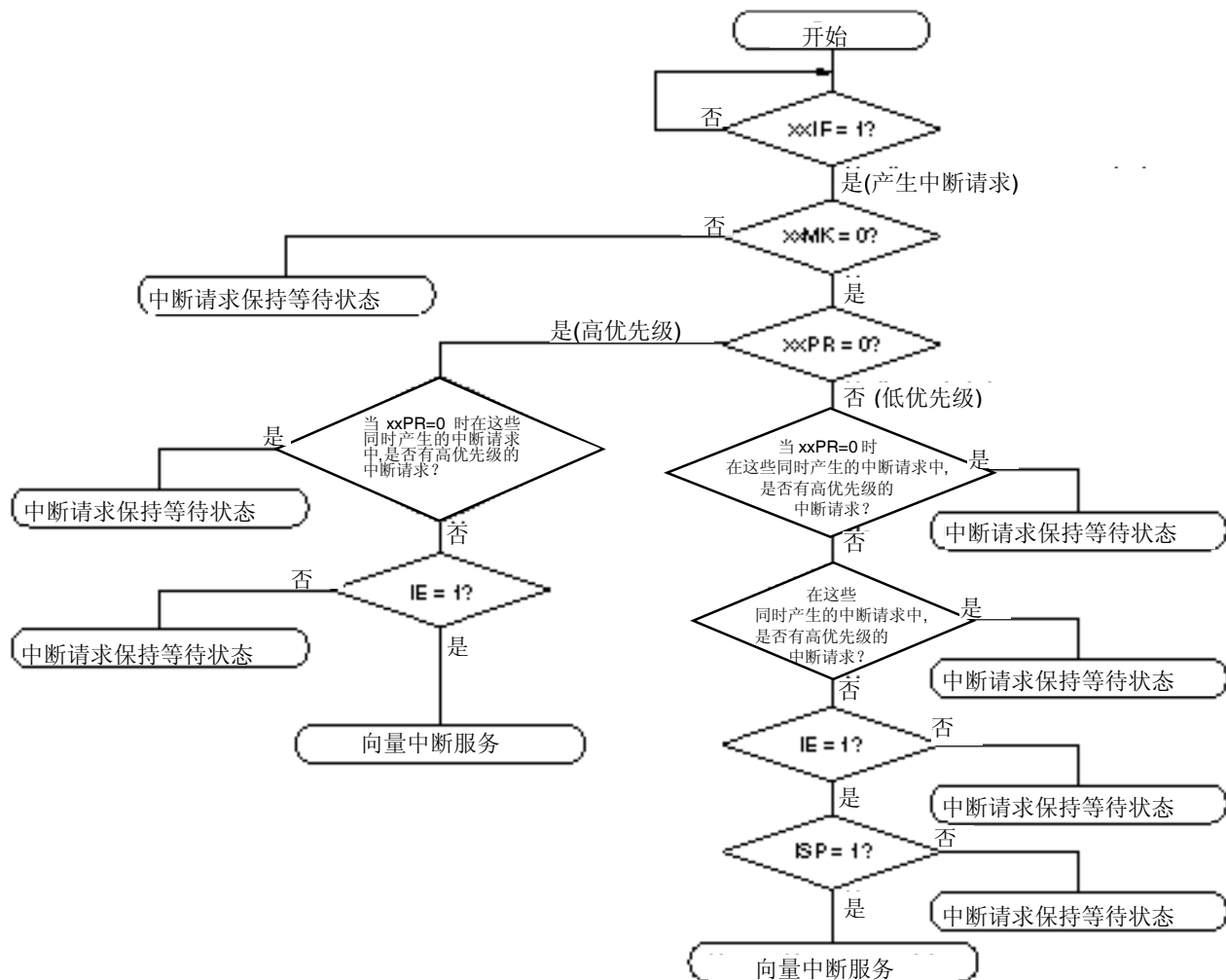
图 20-19. 中断请求响应处理算法
