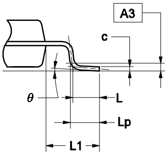
引脚端详图
