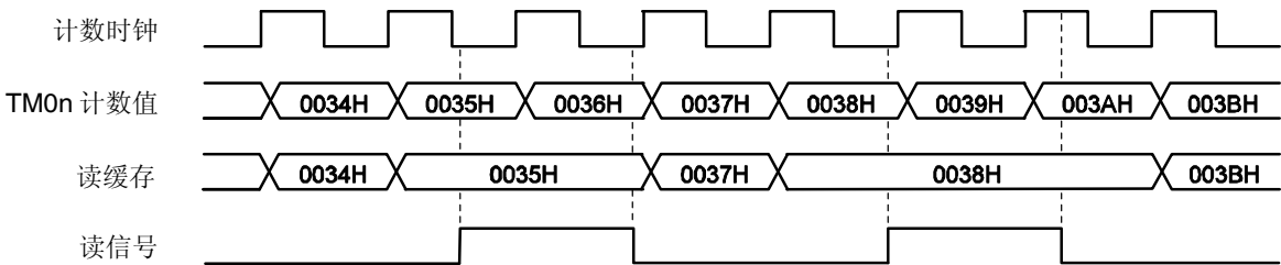
图 7-63. 16 位定时器计数器 0n (TM0n)读取时序
