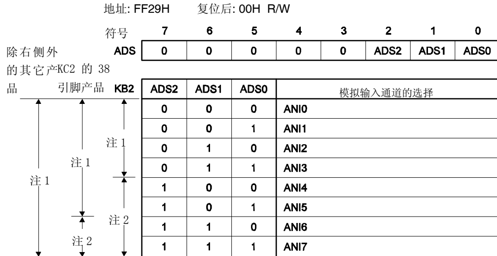
图 13-8. 模拟输入通道选择寄存器 (ADS)的格式
