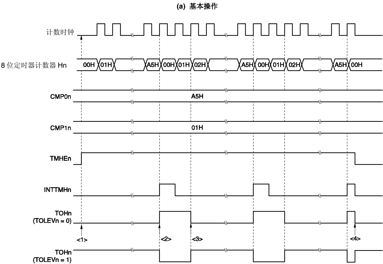
图 9-12 PWM 输出模式下的操作时序(1/4)
