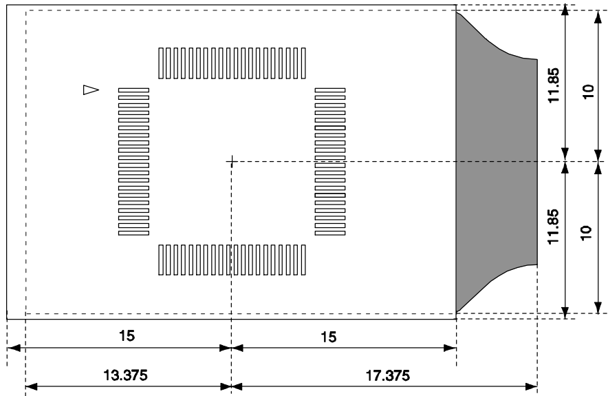
图 B-9. 对于 64 引脚 GC 封装
