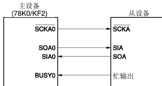
图 17-23 使用忙控制选项时的系统配置
