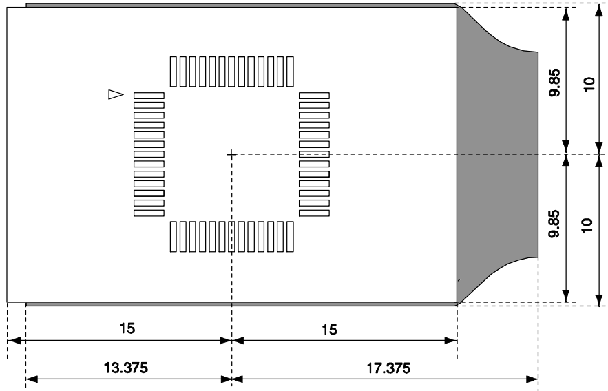
图 B-5. 对于 52 引脚 GB 封装
