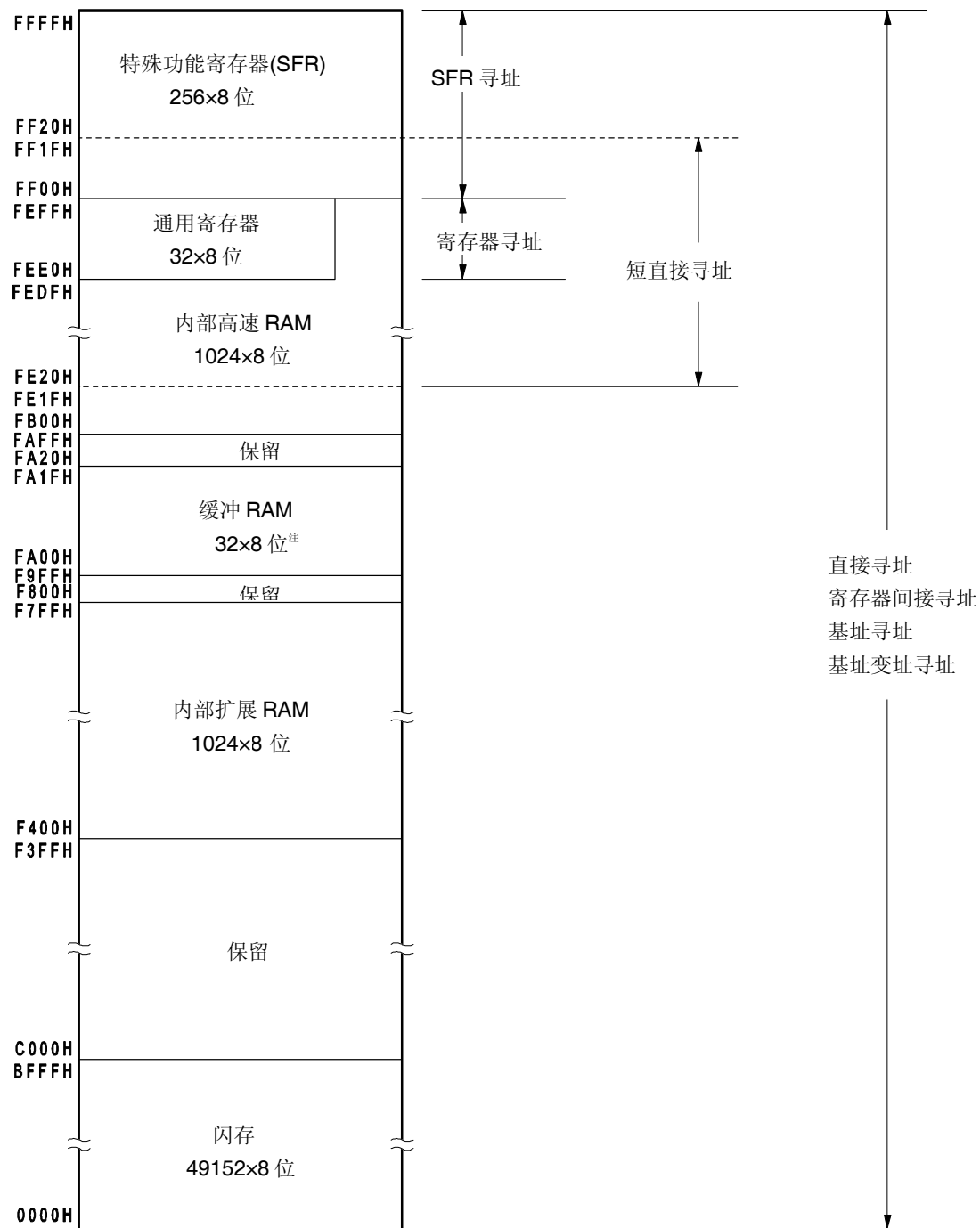
图 3-16. 数据存储空间与寻址方式的对应关系 ( \mu PD78F0514A, 78F0524A, 78F0534A, 78F0544A)
