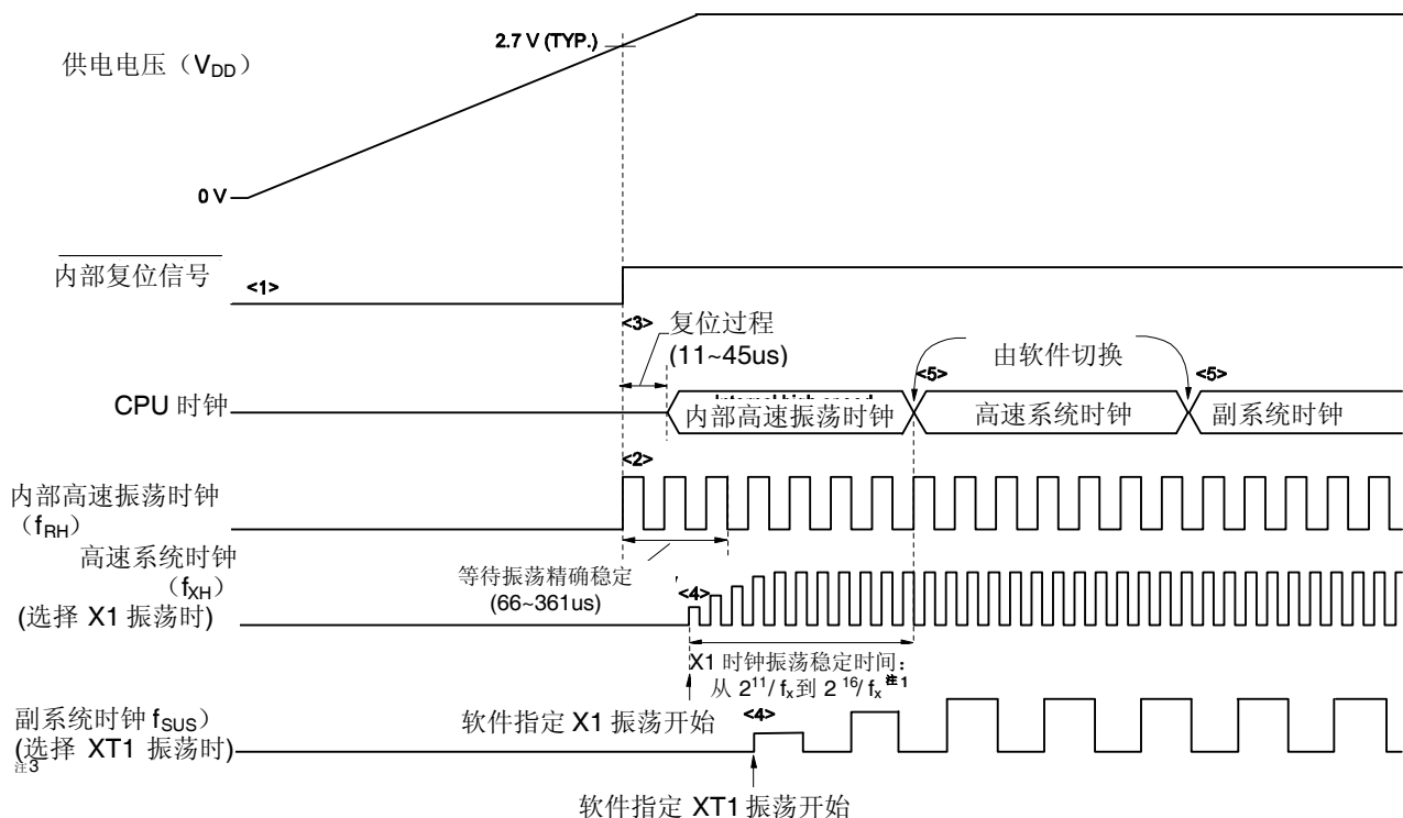
图 6-16. 上电时的时钟发生器操作 (设置 2.7V/1.59V POC 模式(选项字节: POCMODE = 1))
