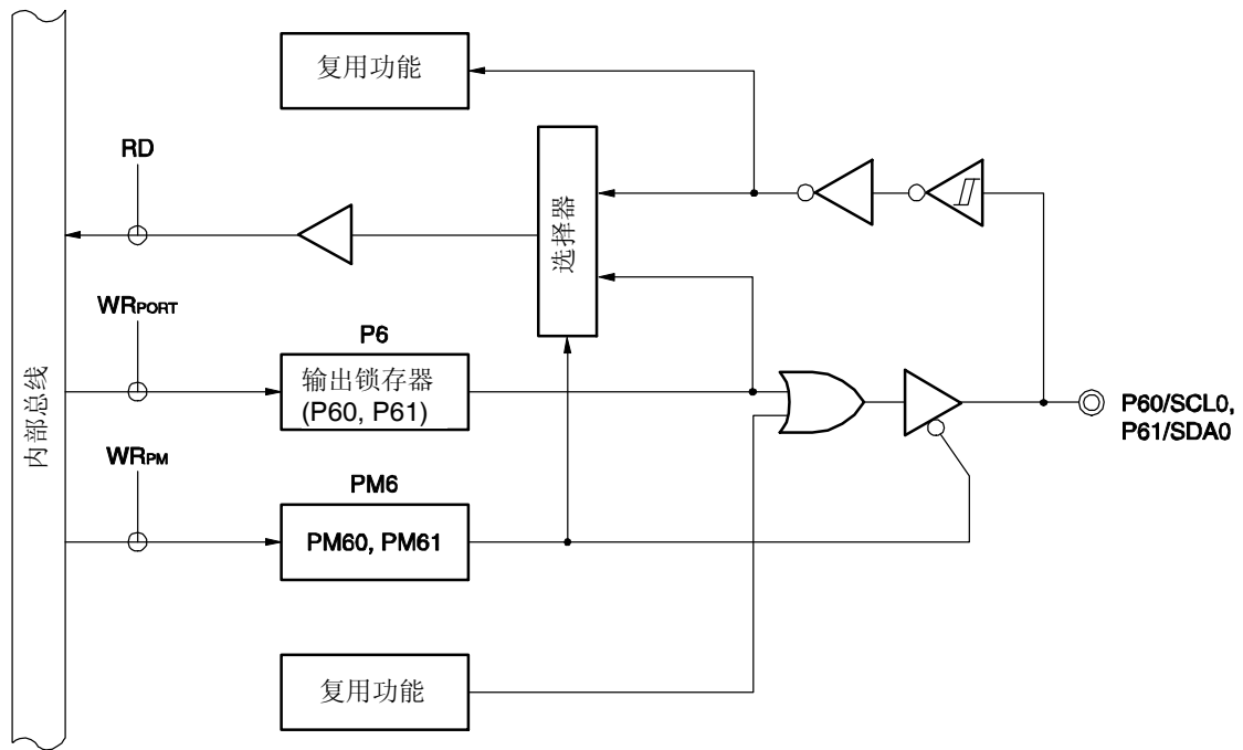
图 5-17. P60 和 P61 的框图
