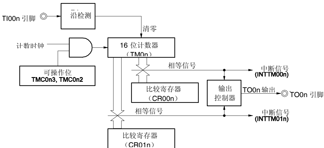
图 7-27 清零&启动模式(通过 TI00n 引脚有效沿输入进入)的框图 (CR00n: 比较寄存器, CR01n: 比较寄存器)
