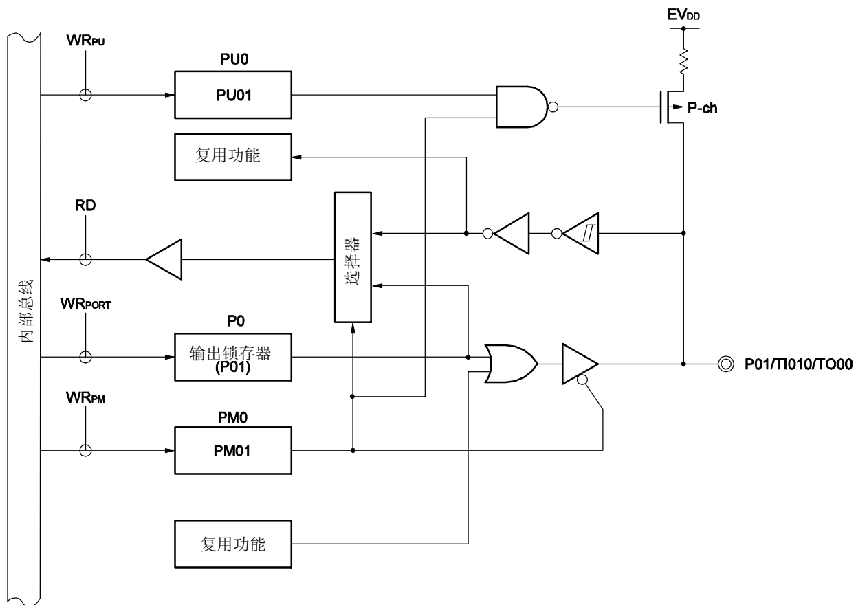
图 5-2. P01 的框图
