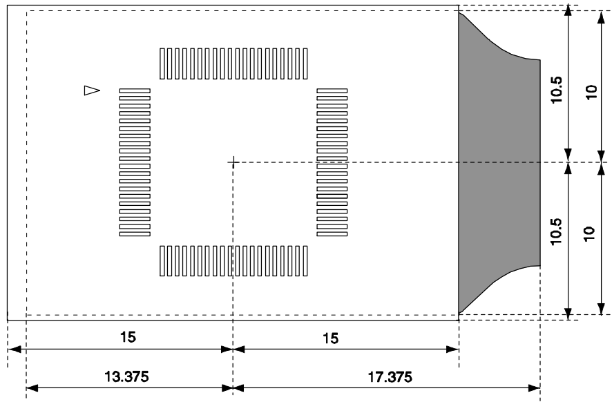
图 B-10. 对于 64 引脚 GK 封装
