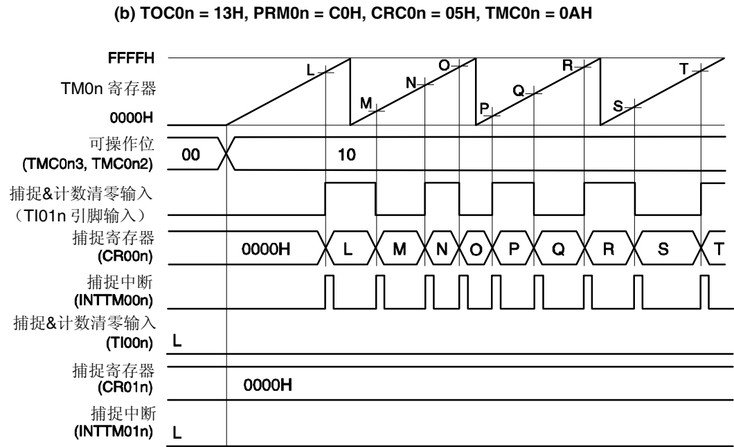
图 7-34 清零&启动模式(通过 TI00n 引脚有效沿输入进入)时序示例 (CR00n: 捕捉寄存器, CR01n: 捕捉寄存器) (2/3)
