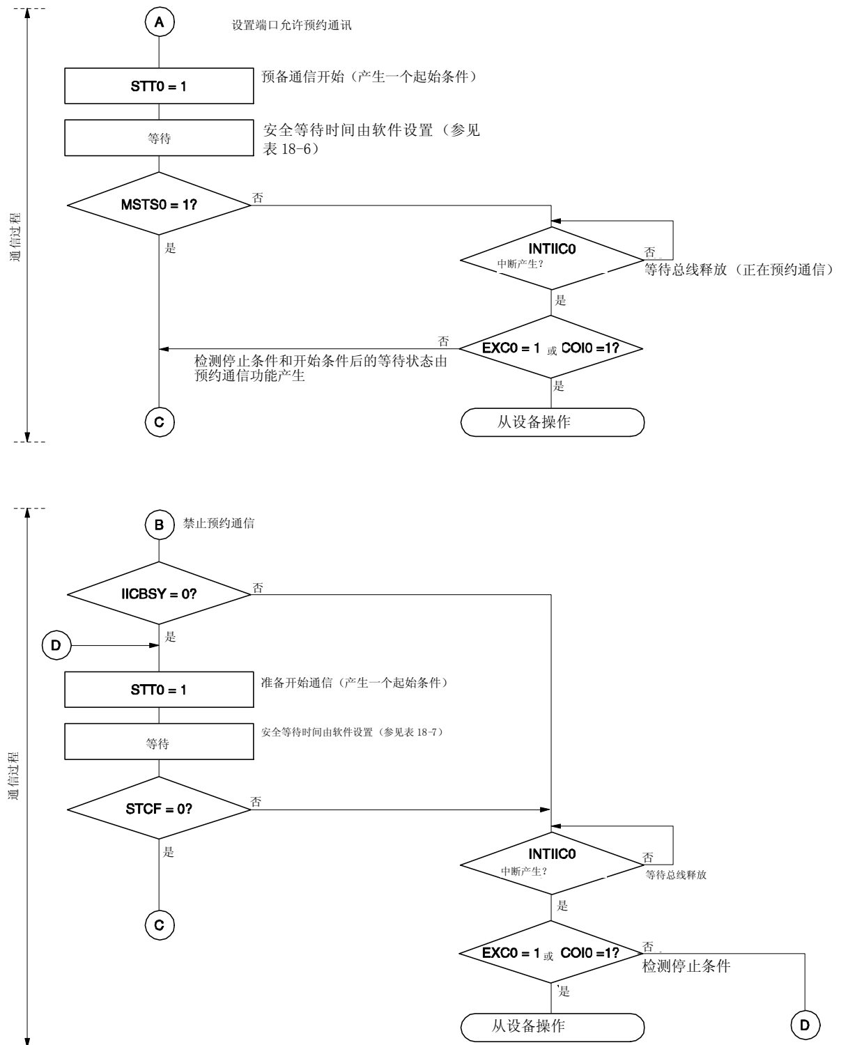
图 18-24. 主设备操作(多主设备系统) (2/3)
