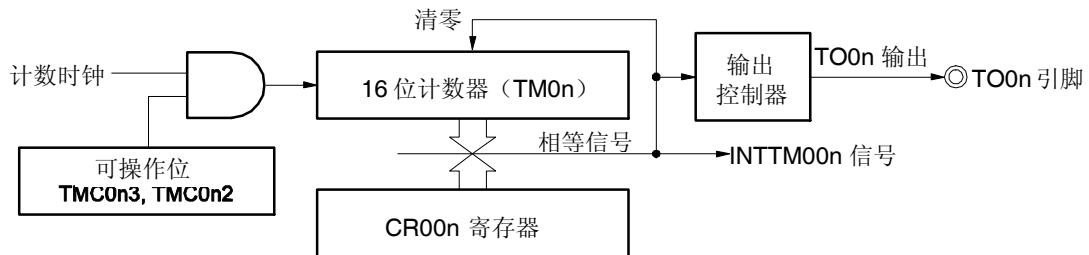
图 7-20 方波输出操作框图
