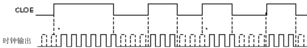
图 12-6. 遥控输出应用举例
