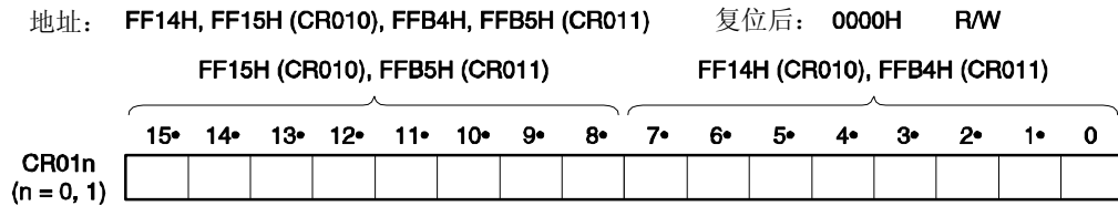
图 7-5.16 16 位定时器捕捉/比较寄存器 01n (CR01n)的格式
