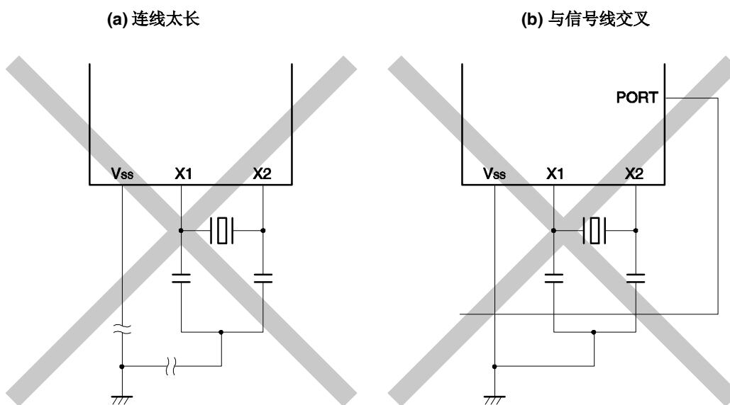
图 6-14. 不正确的振荡器连接示例 (1/2)
