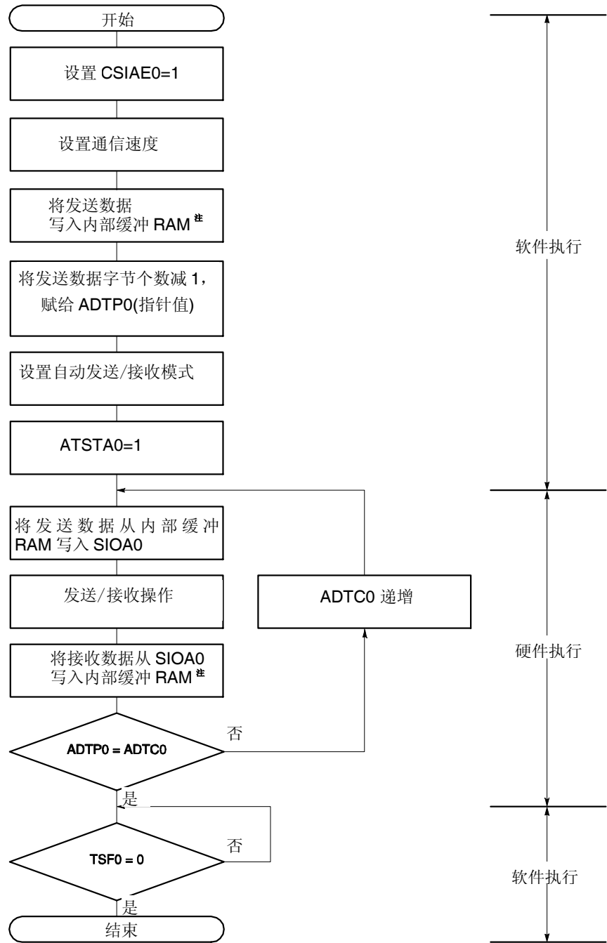
图 17-14 自动发送/接收模式流程图
