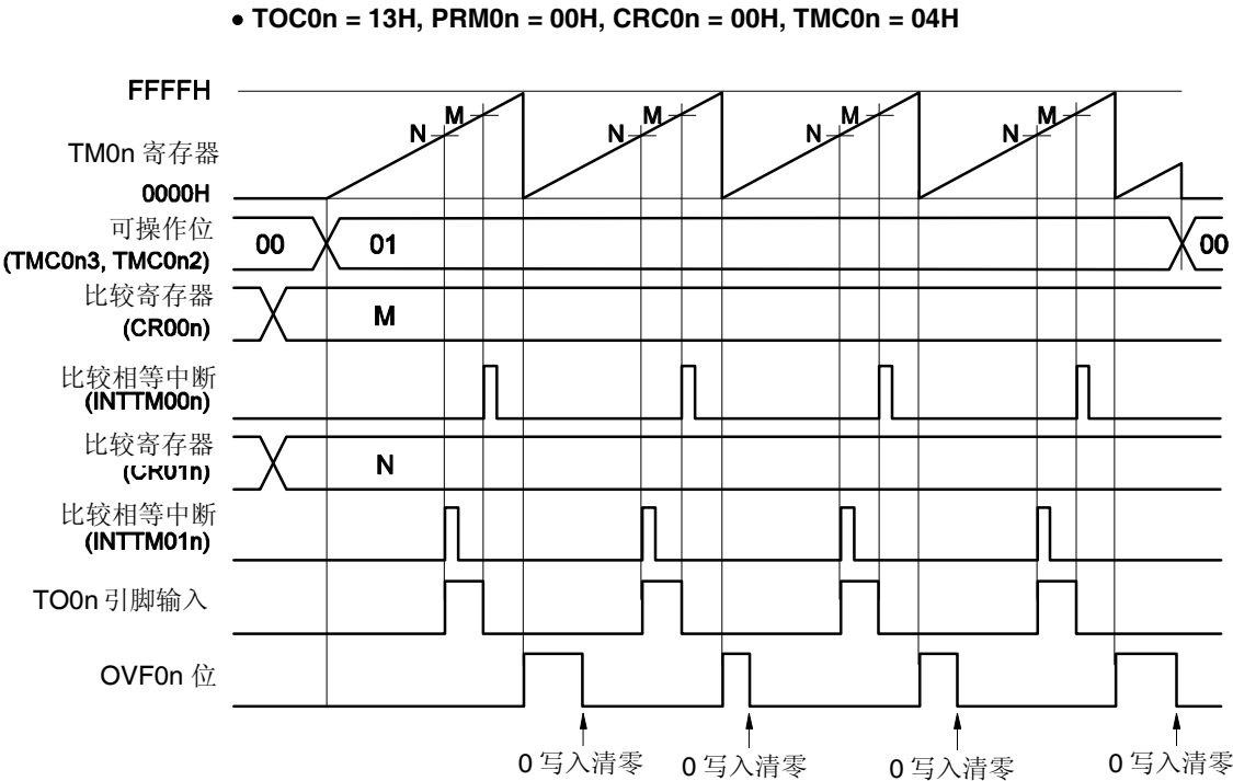
图 7-38 自由运行定时器模式时序示例 (CR00n: 比较寄存器, CR01n: 比较寄存器)
