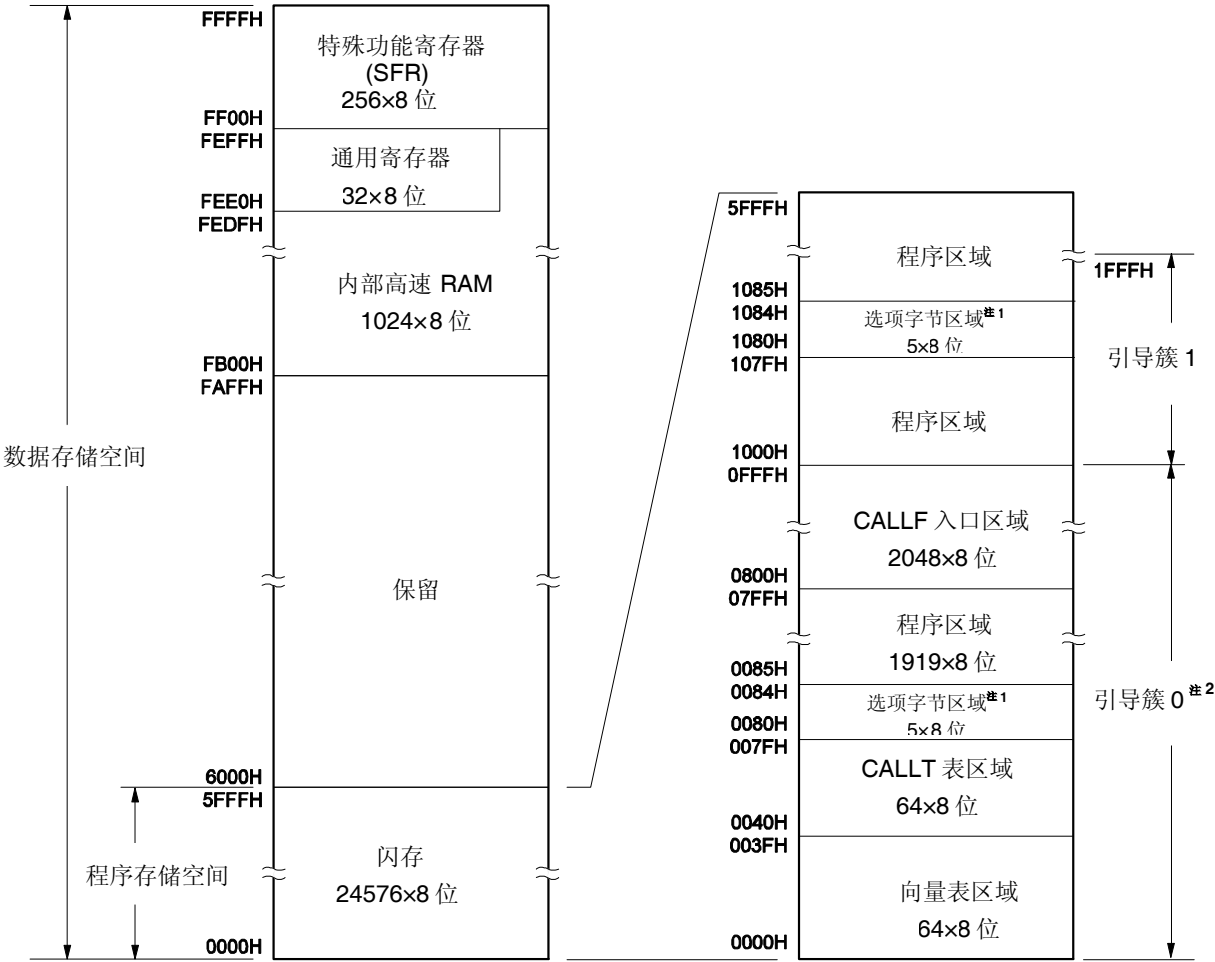
图 3-3. 存储空间映射图 (μPD78F0502A, 78F0512A, 78F0522A, 78F0532A)
