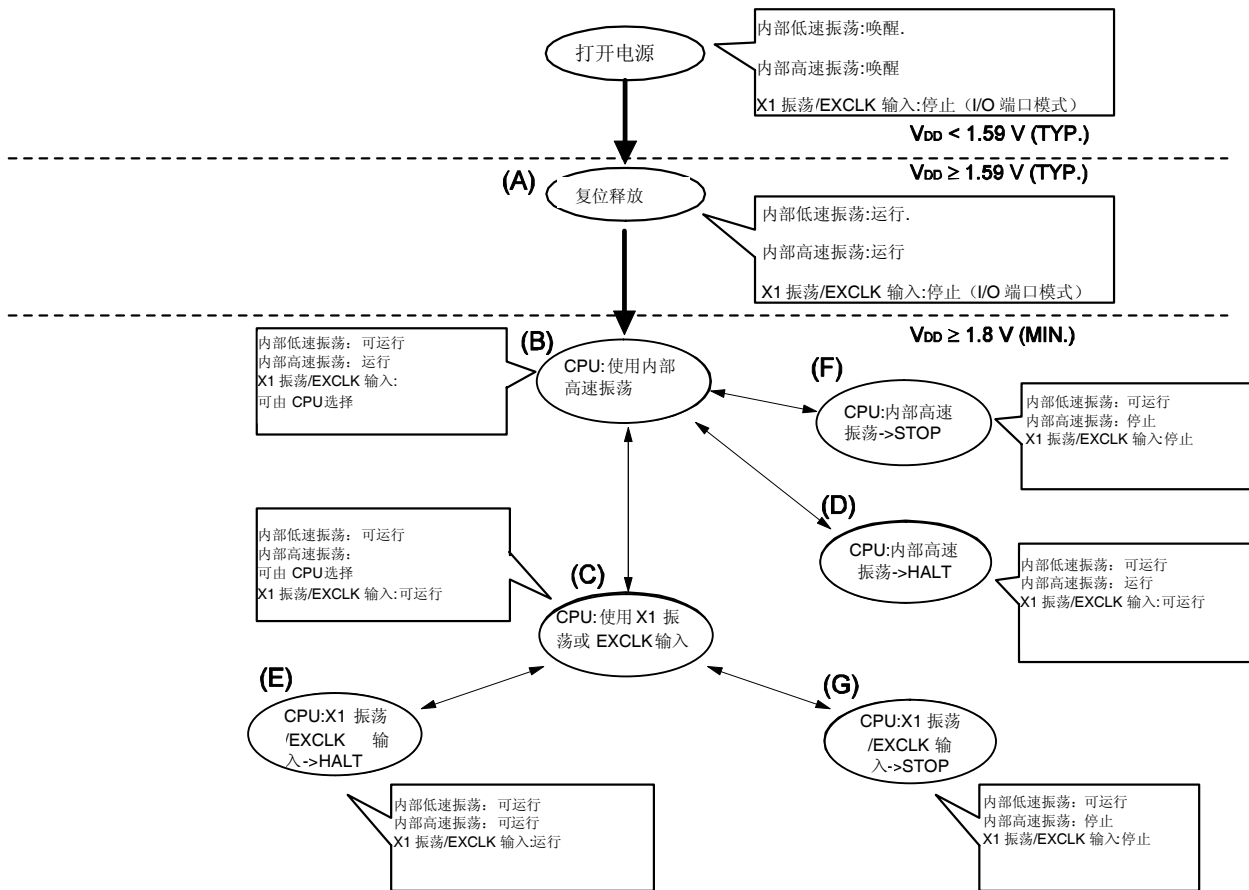
图 6-17. CPU 时钟状态转移图 (设置 1.59 V POC 模式 (选项字节: POCMODE = 0), 78K0/KB2)
