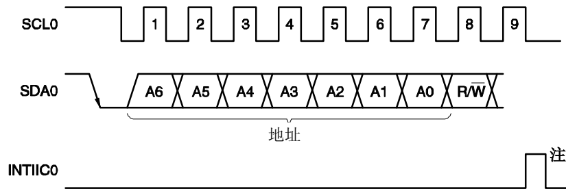
图 18-14. 地址
