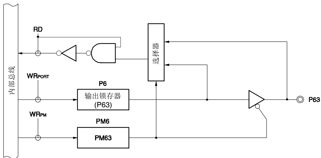
图 5-19. P63 的框图
