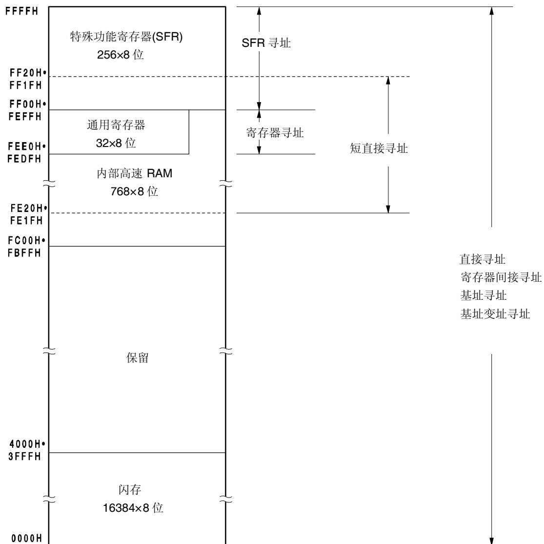
图 3-13. 数据存储空间与寻址方式的对应关系 ( \mu PD78F0501A, 78F0511A, 78F0521A,和 78F0531A)
