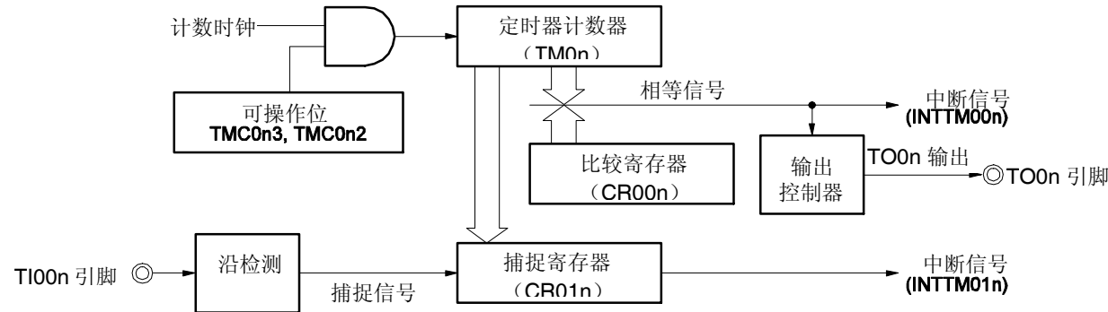
图 7-39 自由运行定时器模式的框图 (CR00n: 比较寄存器, CR01n: 捕捉寄存器)
