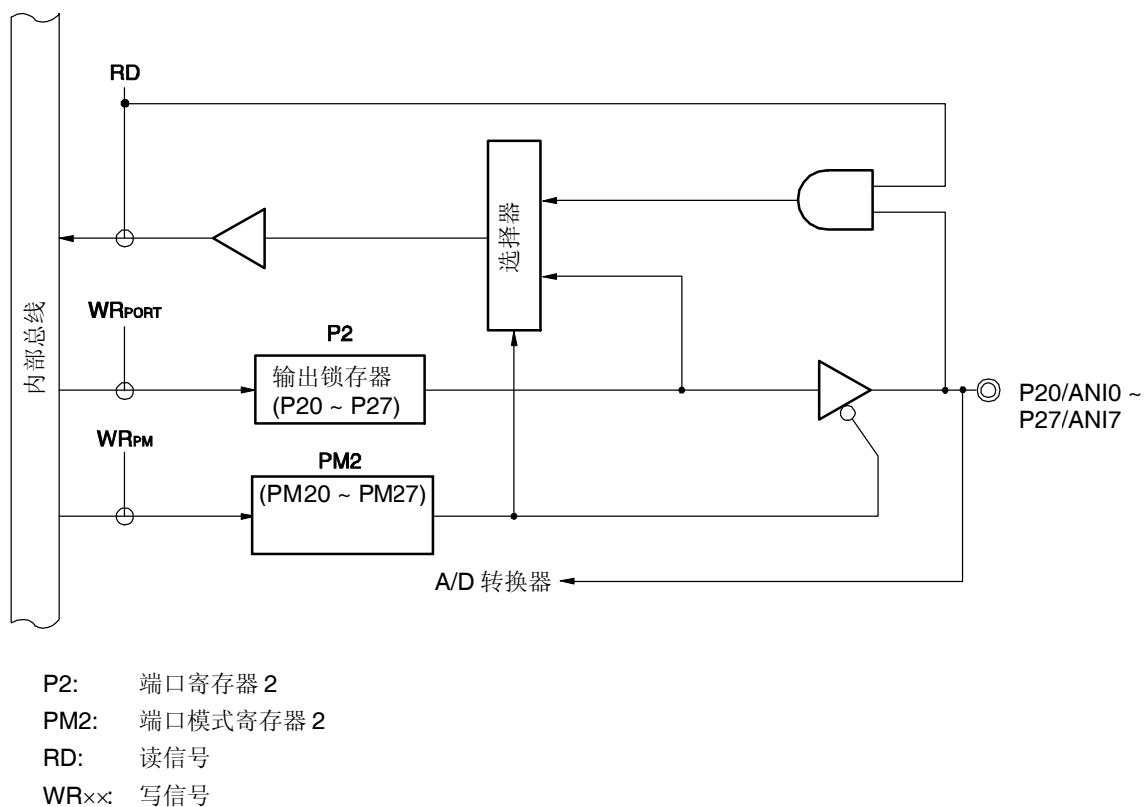
图 5-12. P20 ~ P27 的框图
