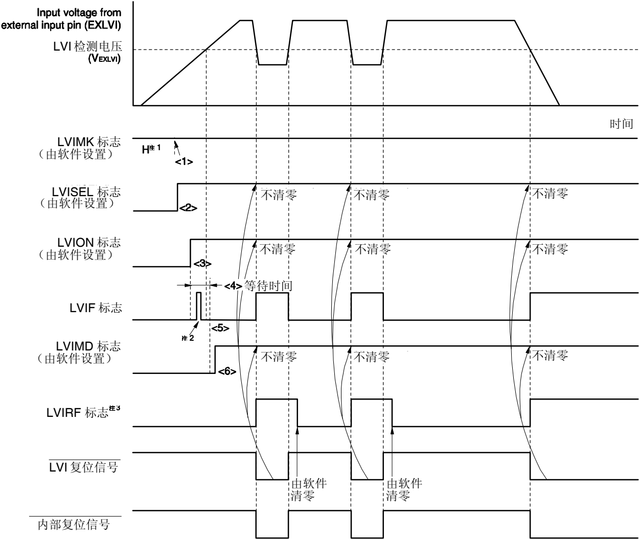
图 25-6. 低电压检测电路内部复位信号的产生时序 (检测外部输入引脚(EXLVI)的输入电压的等级)
