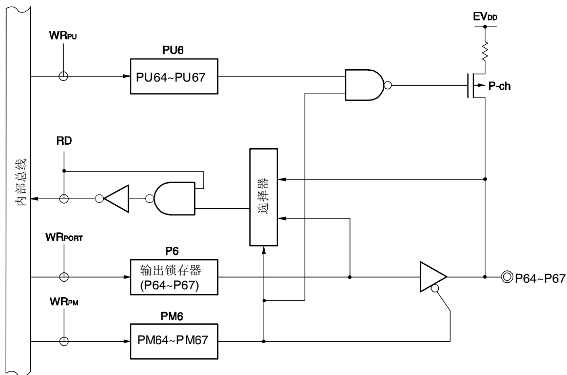
图 5-20. P64~P67 的框图
