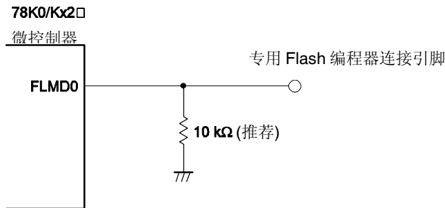
图 27-6. FLMD0 引脚连接示例
