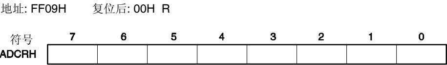
图 13-7 8 位 A/D 转换结果寄存器(ADCRH) 的格式
