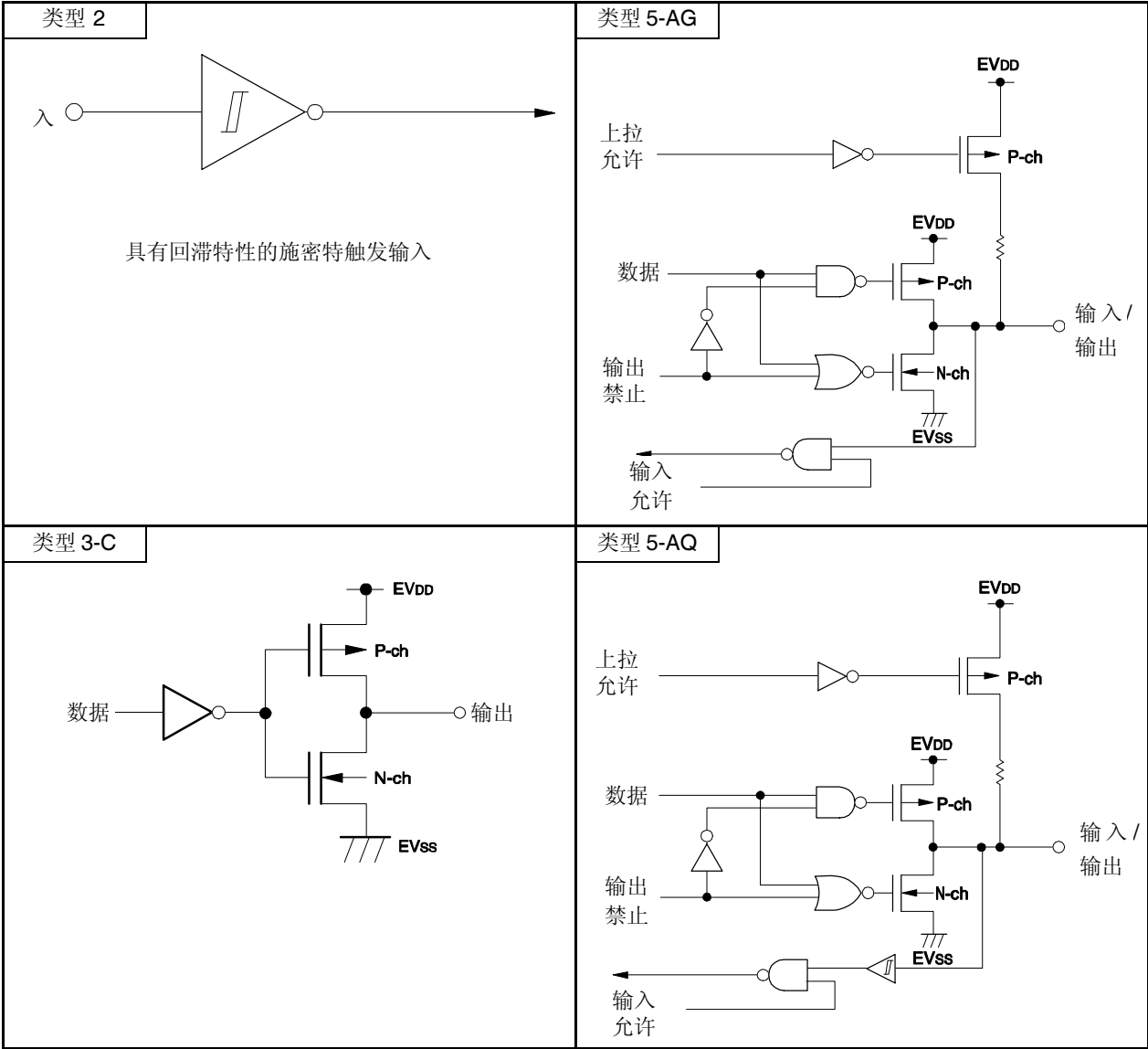
图 2-1. 引脚 I/O 电路列表(1/2)
