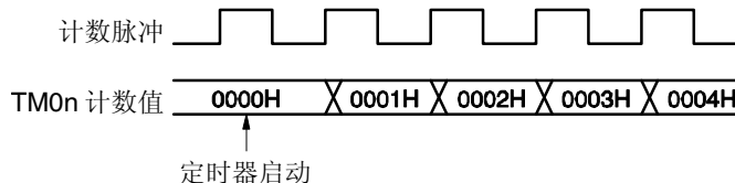
图 7-60. TM0n 计数启动时序
