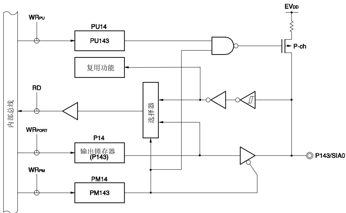
图 5-27. 的框图 P143
