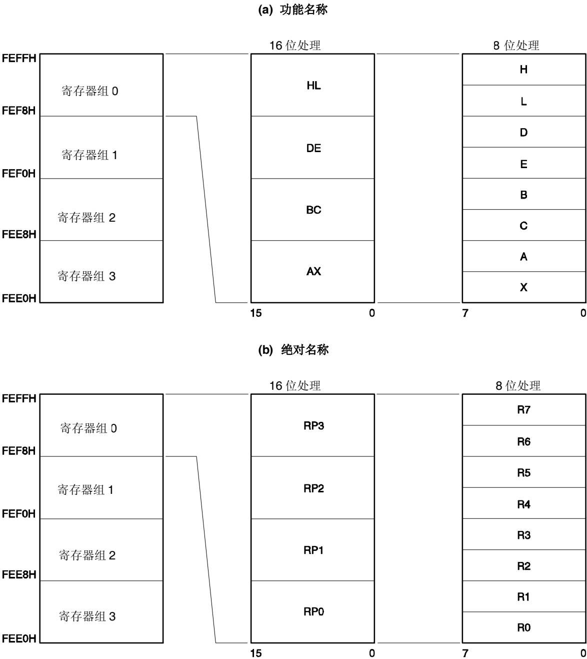
图 3-25. 通用寄存器结构
