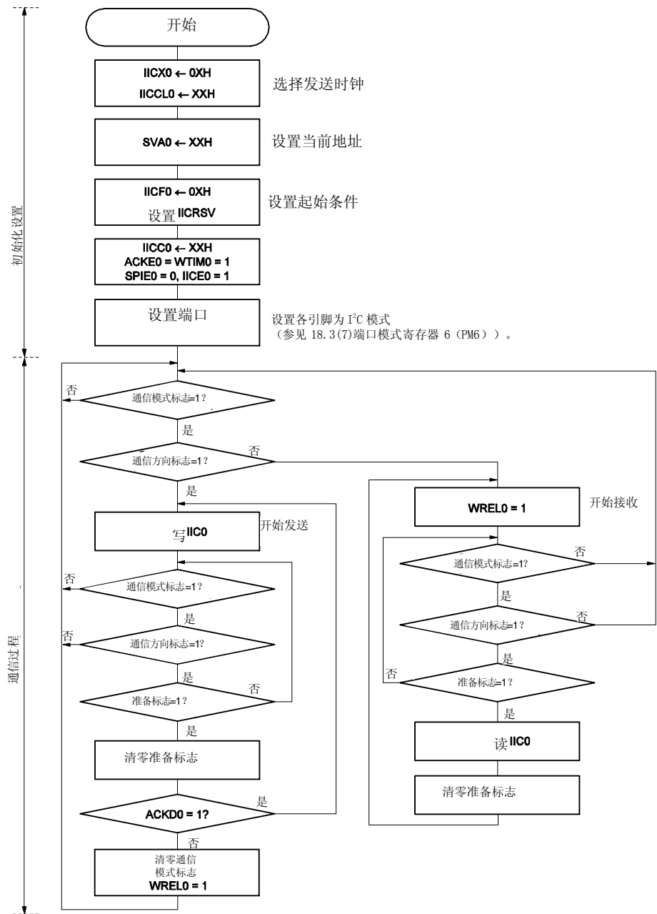
图 18-25. 从设备操作流程(1)
