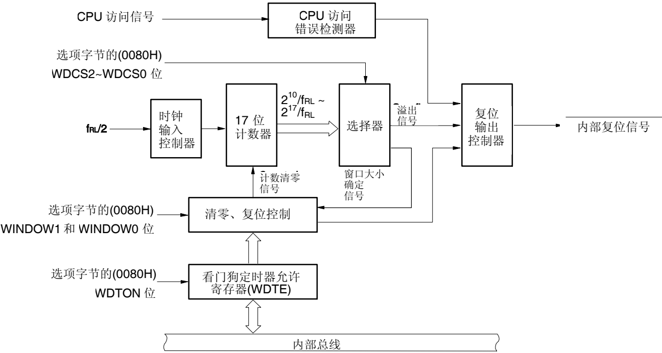
图 11-1 看门狗定时器的框图
