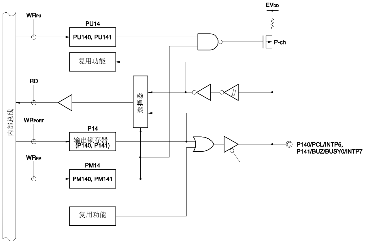
图 5-25. P140 和 P141 的框图
