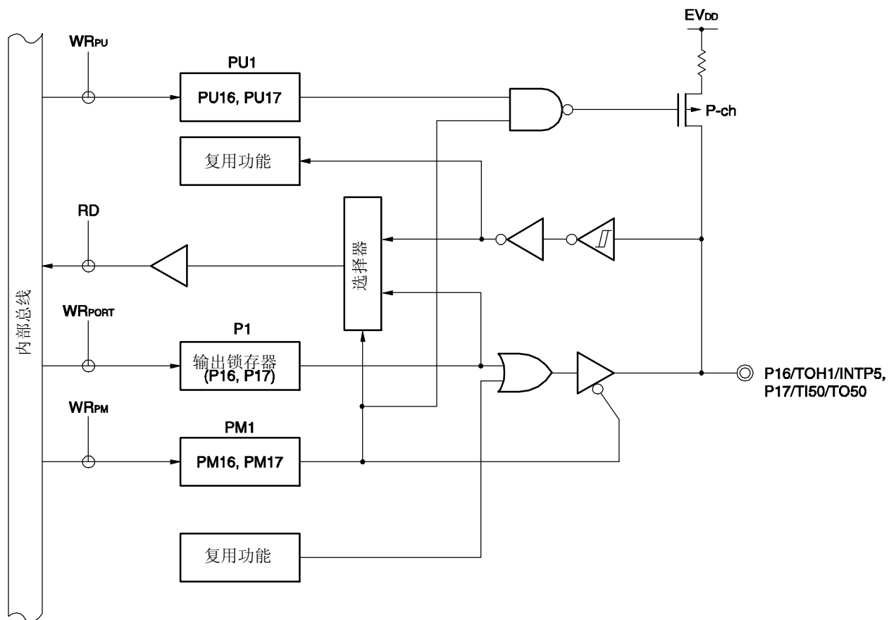
图 5-11. P16 和 P17 的框图
