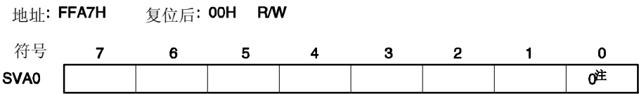
图 18-4. 从地址寄存器 0 的格式 (SVA0)
