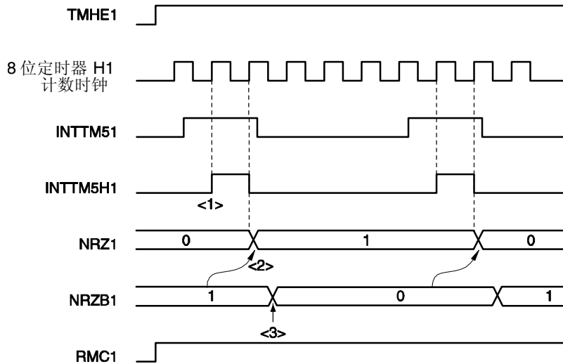
图 9-13 传送时序
