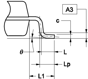
引脚端详图
