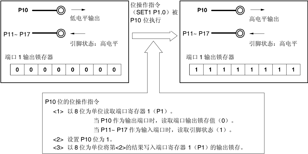
图 5-45. 位操作指令(P10)
