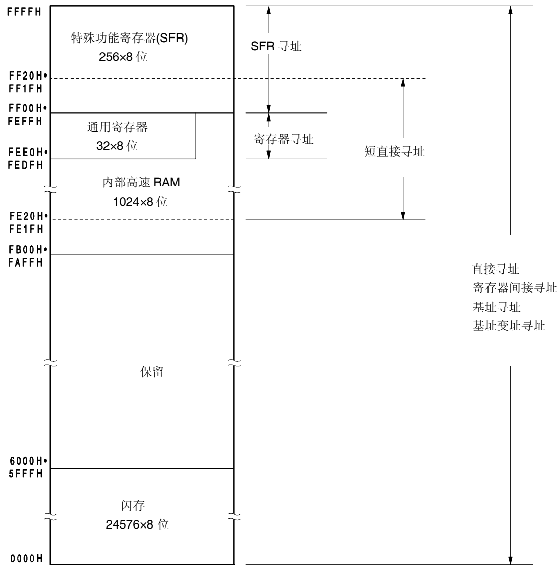
图 3-14. 数据存储空间与寻址方式的对应关系 ( \mu PD78F0502A, 78F0512A, 78F0522A, 78F0532A)
