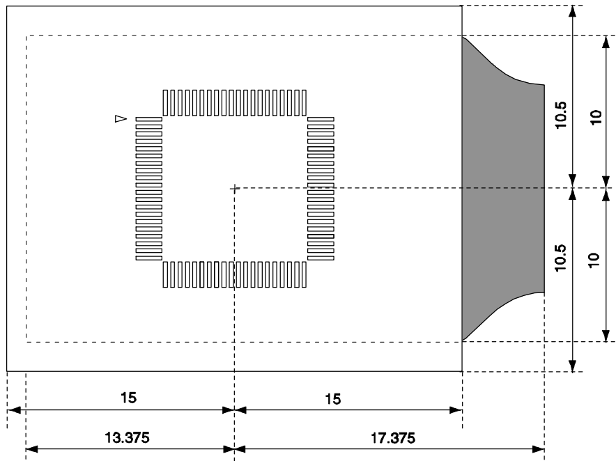
图 B-8. 对于 64 引脚 GB 封装
