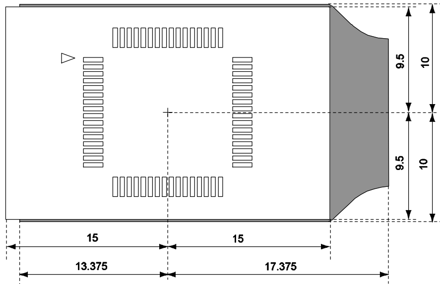
图 B-7. 对于 64 引脚 GA 封装
