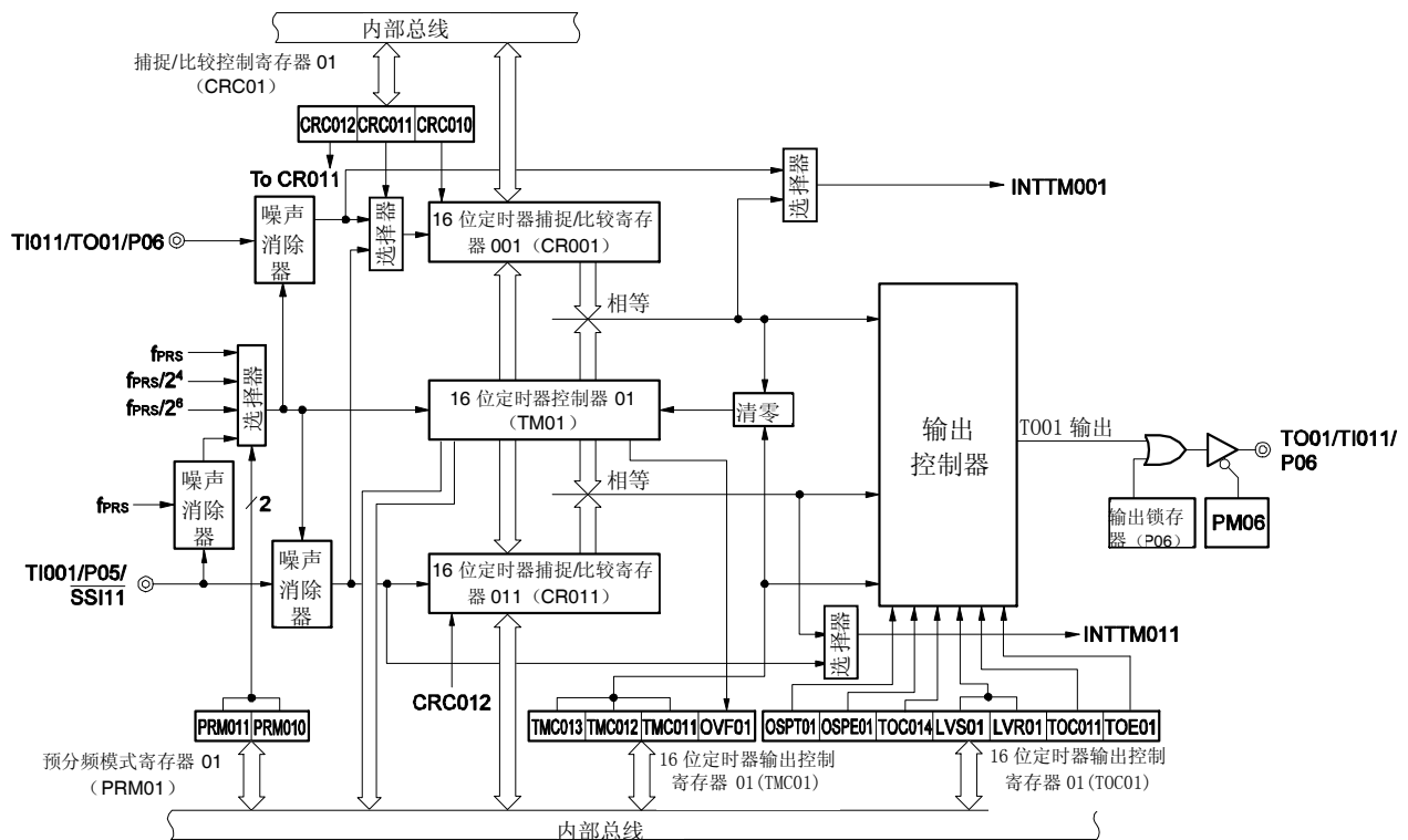
图 7-2. 16 位定时器/事件计数器 01 的框图
