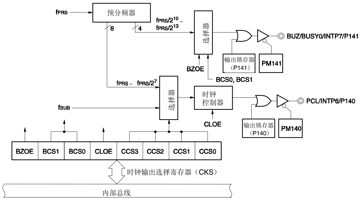
图 12-2. 时钟输出/蜂鸣器输出控制器的框图(78K0/KE2, 78K0/KF2)
