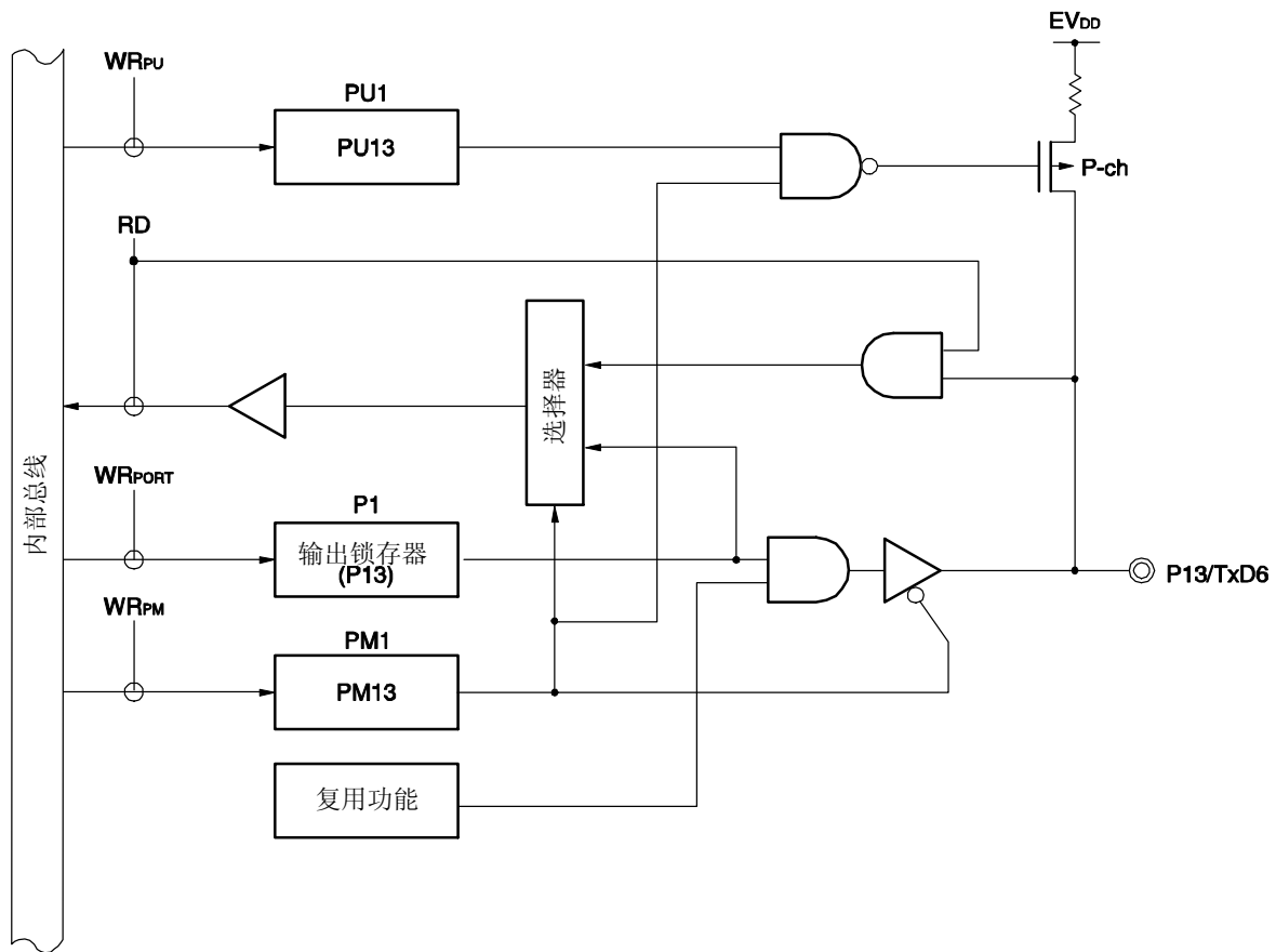
图 5-10. P13 的框图
