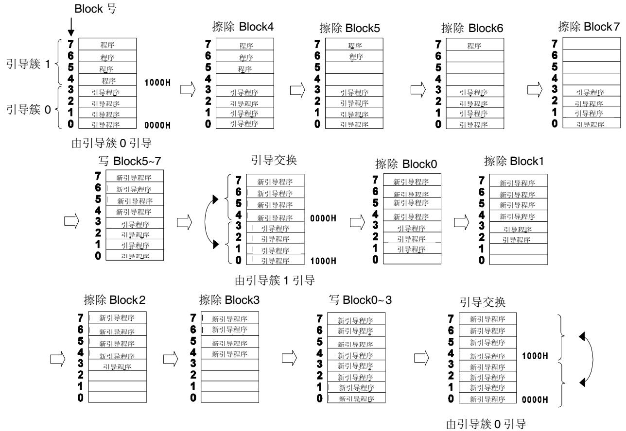
图 27-16. 执行引导交换的示例
