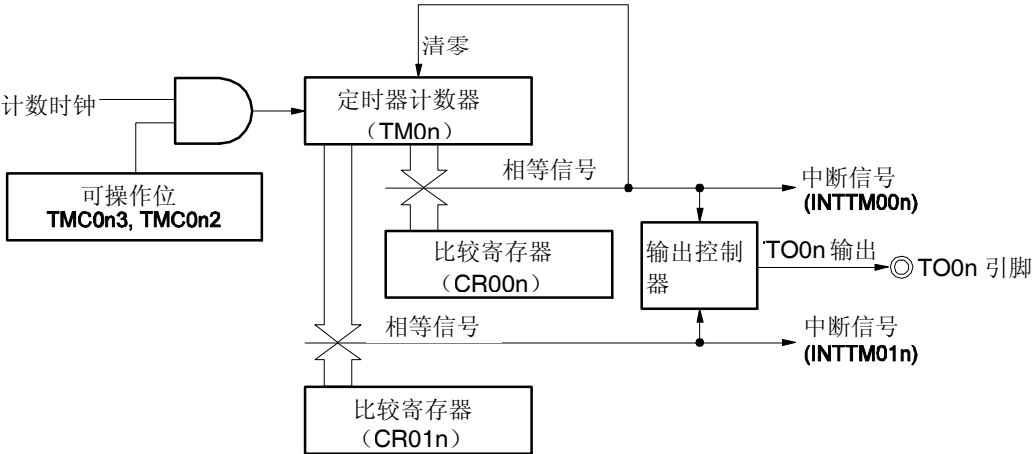
图 7-45 PPG 输出操作的框图
