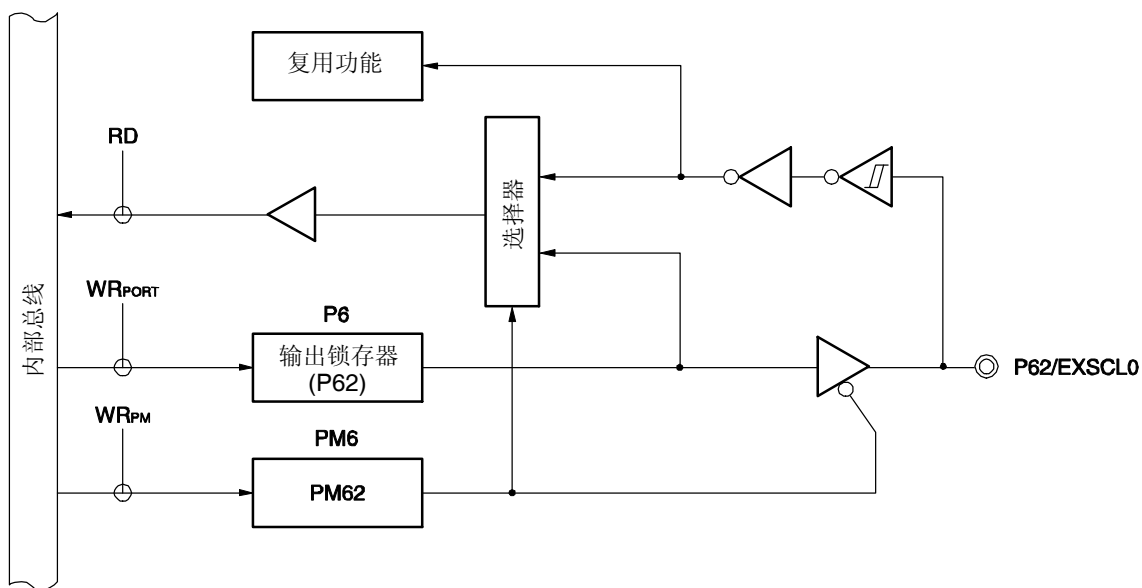
图 5-18. P62 的框图
