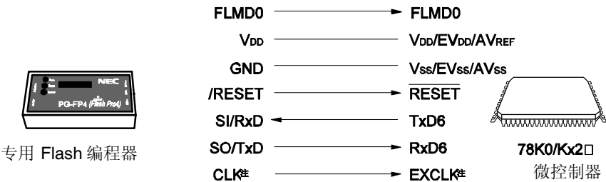
图 27-5. 专用 Flash 编程器的通信(UART6)
