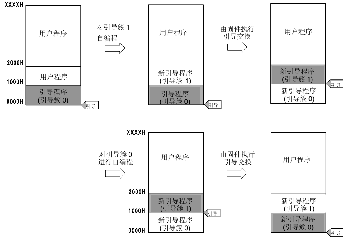
图 27-15. 引导交换功能
