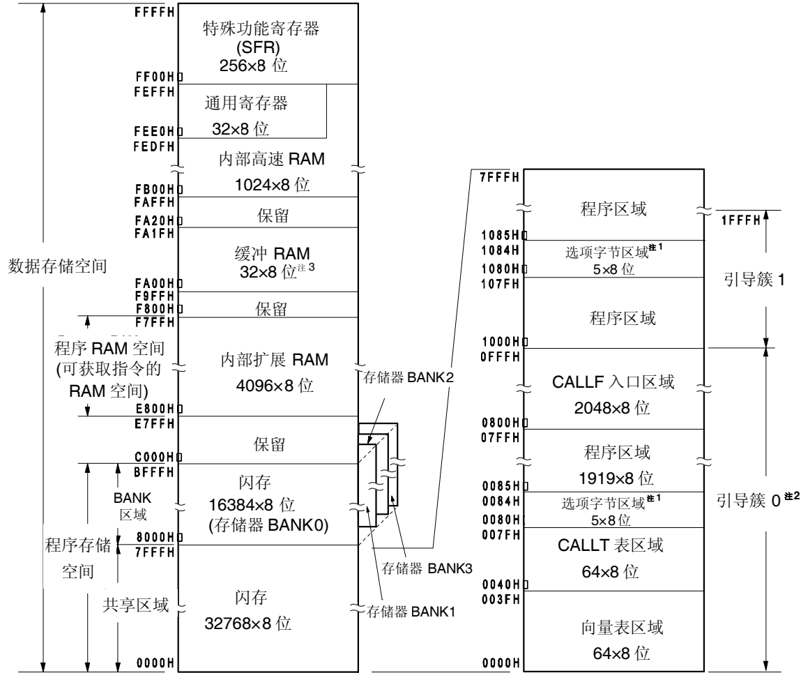
图 3-9. 存储空间映射图 (μPD78F0526A, 78F0536A, 78F0546A)
