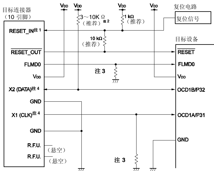
图 28-2. QB-78K0MINI 或 QB-MINI2 与 \mu PD78F05xxDA 的连接示例 (当使用 OCD1A/P31 和 OCD1B/P32 时)
