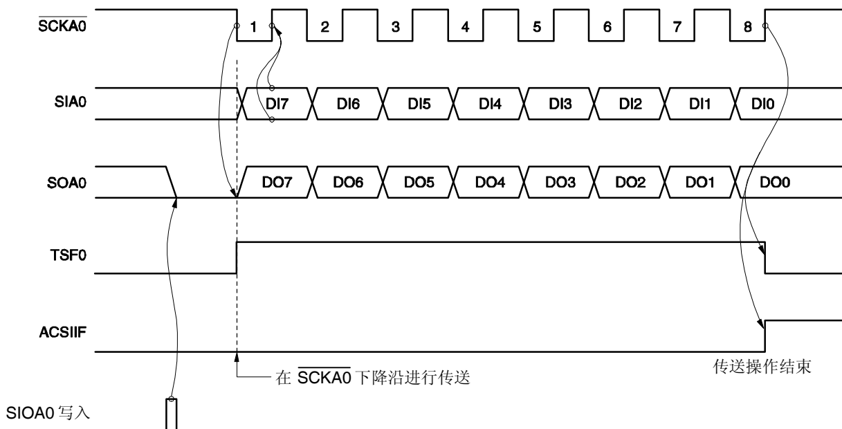
图 17-10 3 线串行 I/O 模式的时序
