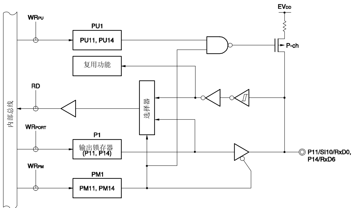
图 5-8. P11 和 P14 的框图
