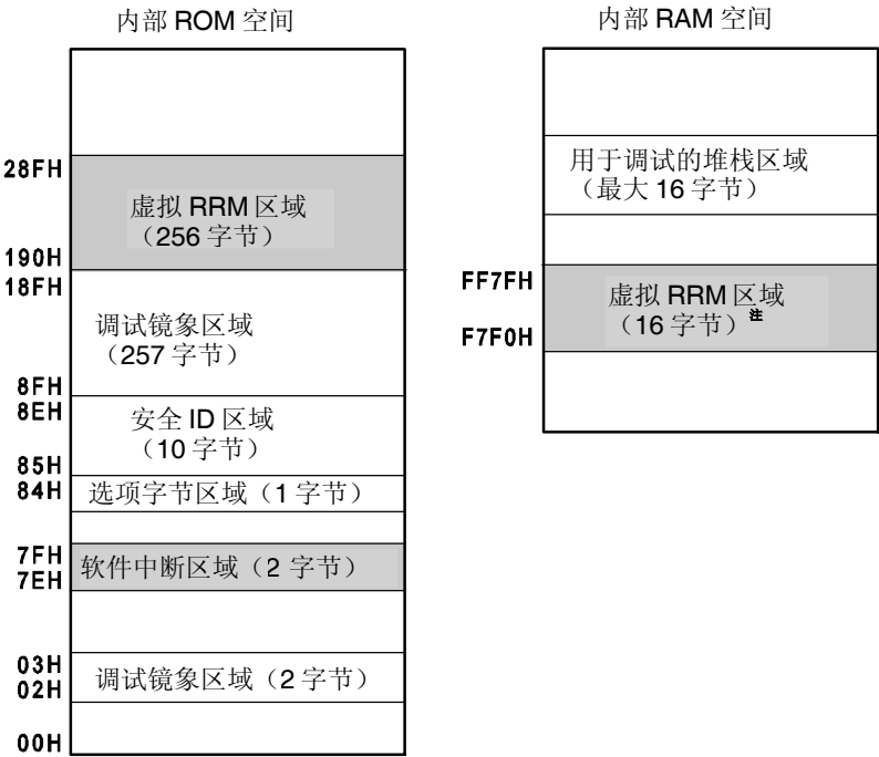
图 28-4. 由 QB-78K0MINI 和 QB-MINI2 使用的保留区域
