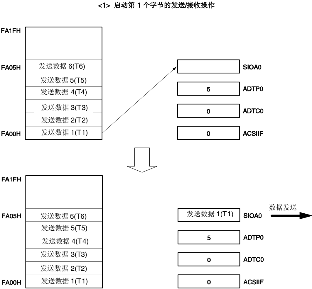
图 17-15 在自动发送/接收模式下内部缓冲 RAM 的操作 (启动发送/接收) (1/2)
