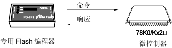
图 27-12. 通信命令
