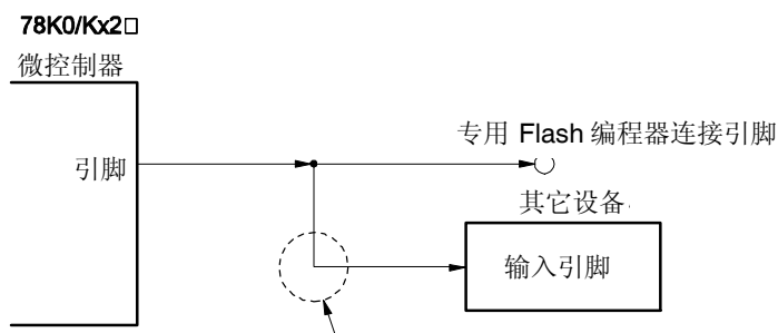
图 27-8. 其它设备的故障
