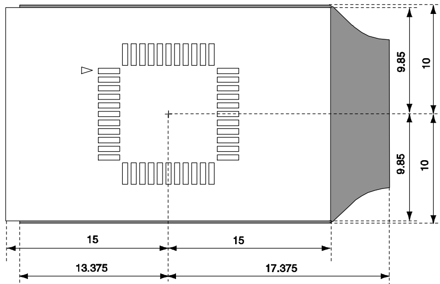
图 B-3. 对于 44 引脚 GB 封装
