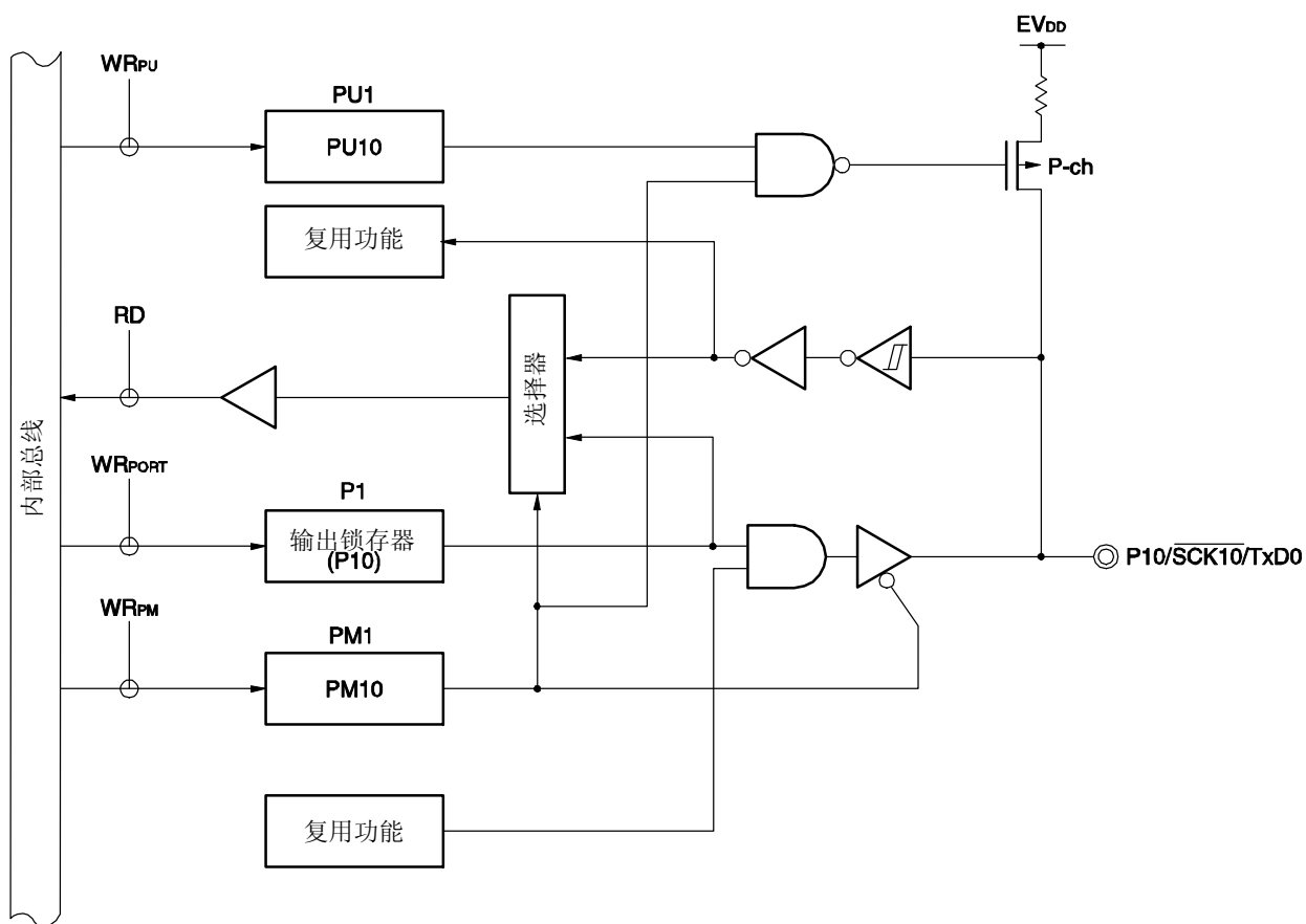
图 5-7. P10 的框图
