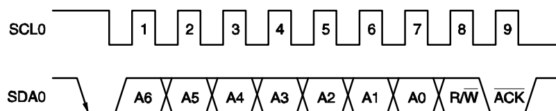
图 18-16. ACK
