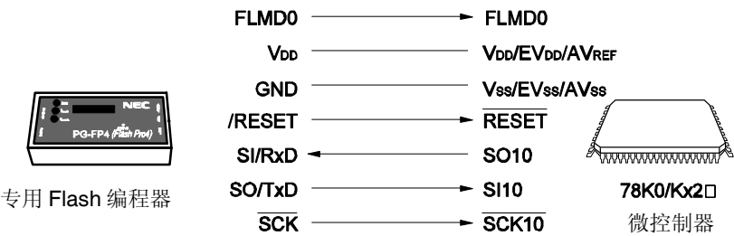
图 27-4. 专用 Flash 存储器编程器的通信（CSI10）
