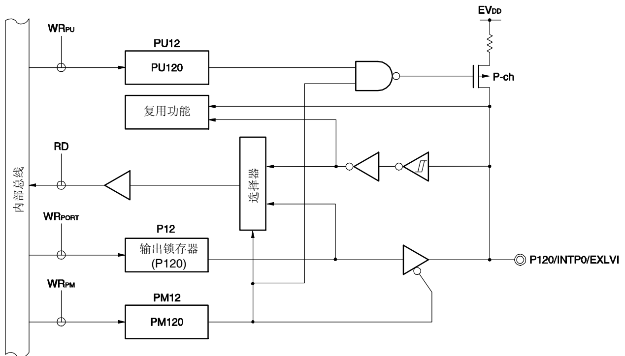
图 5-22. P120 的框图
