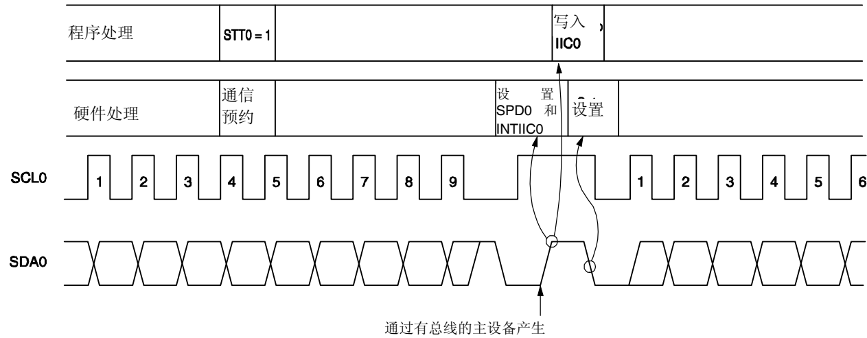
图 18-20. 通信预约时序
