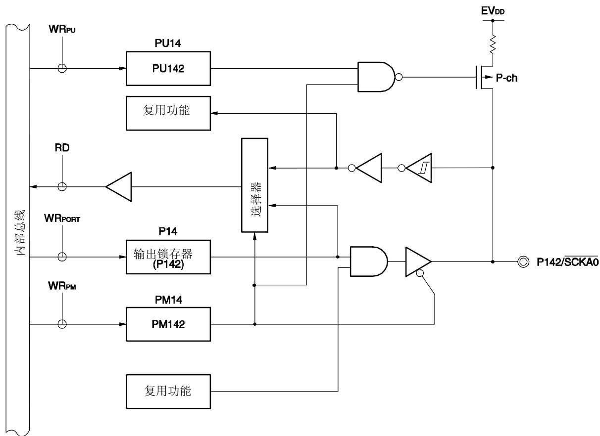
图 5-26. P142 的框图
