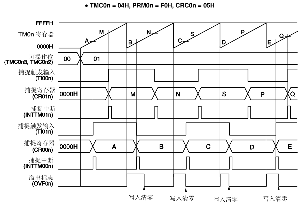
图 7-53. 脉冲宽度测量时序示例(1)
