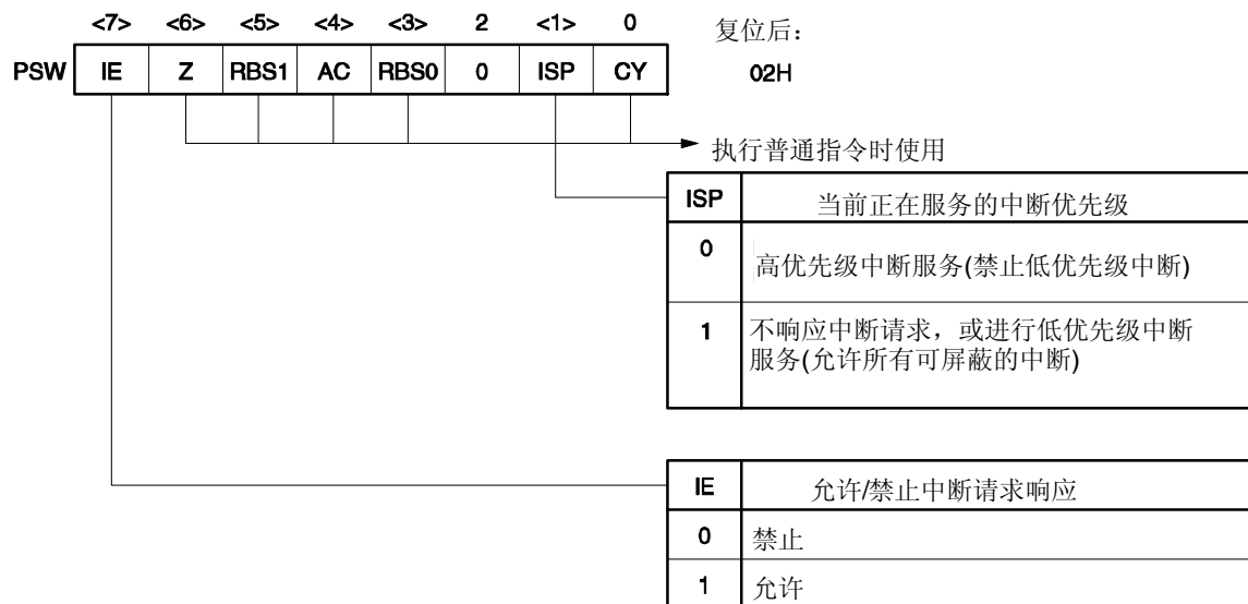
图 20-18. 程序状态字的格式
