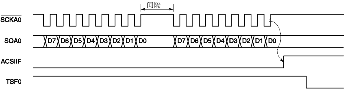
图 17-17 自动发送模式操作时序
