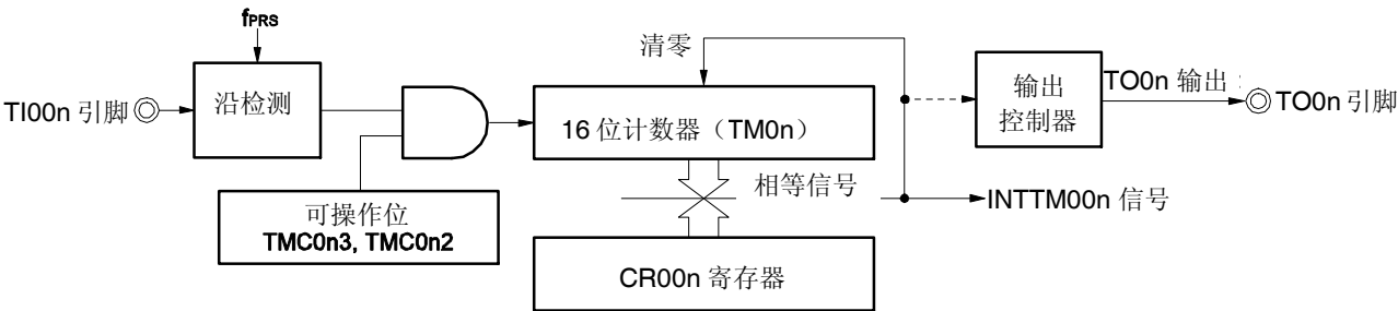
图 7-24 外部事件计数器操作框图
