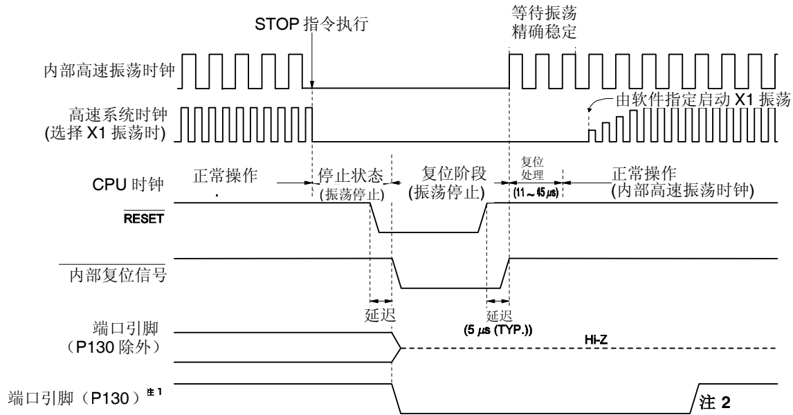
图 23-4. 在 STOP 模式下通过 RESET 输入进行复位的时序
