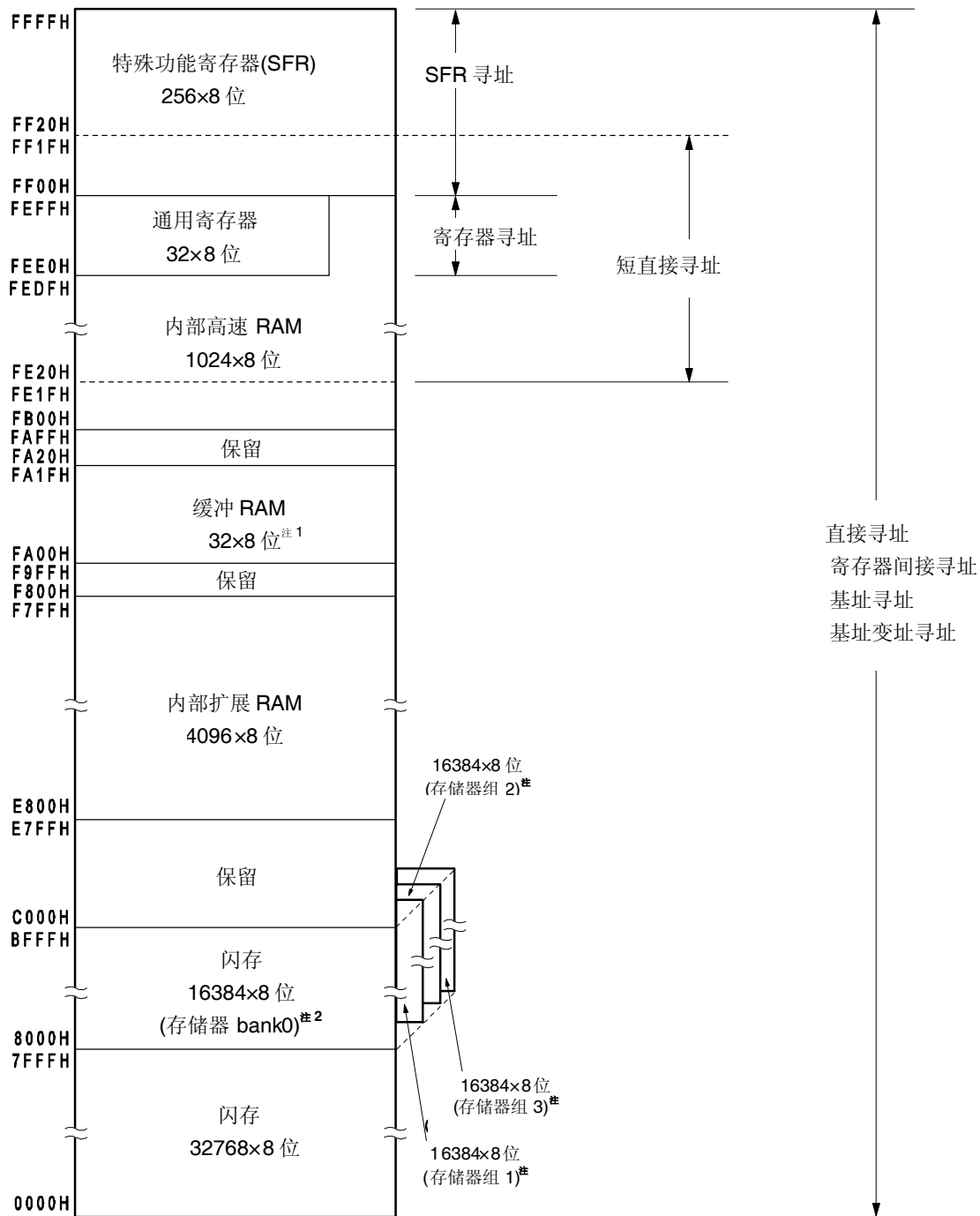
图 3-18. 数据存储空间与寻址方式的对应关系 (μPD78F0526A, 78F0536A, 78F0546A)
