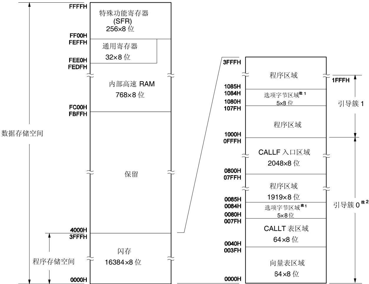
图 3-2. 存储空间映射图 (μPD78F0501A, 78F0511A, 78F0521A, 78F0531A)
