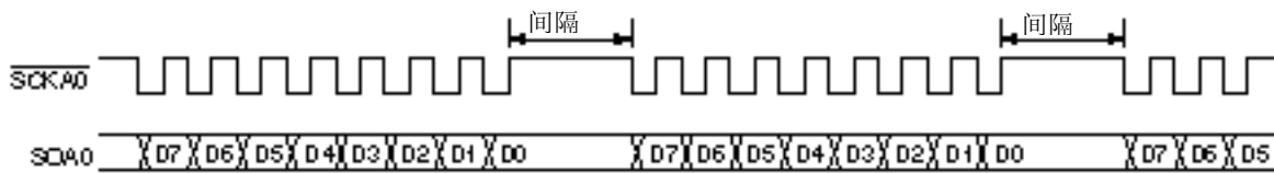
图 17-19 重复发送模式操作时序
