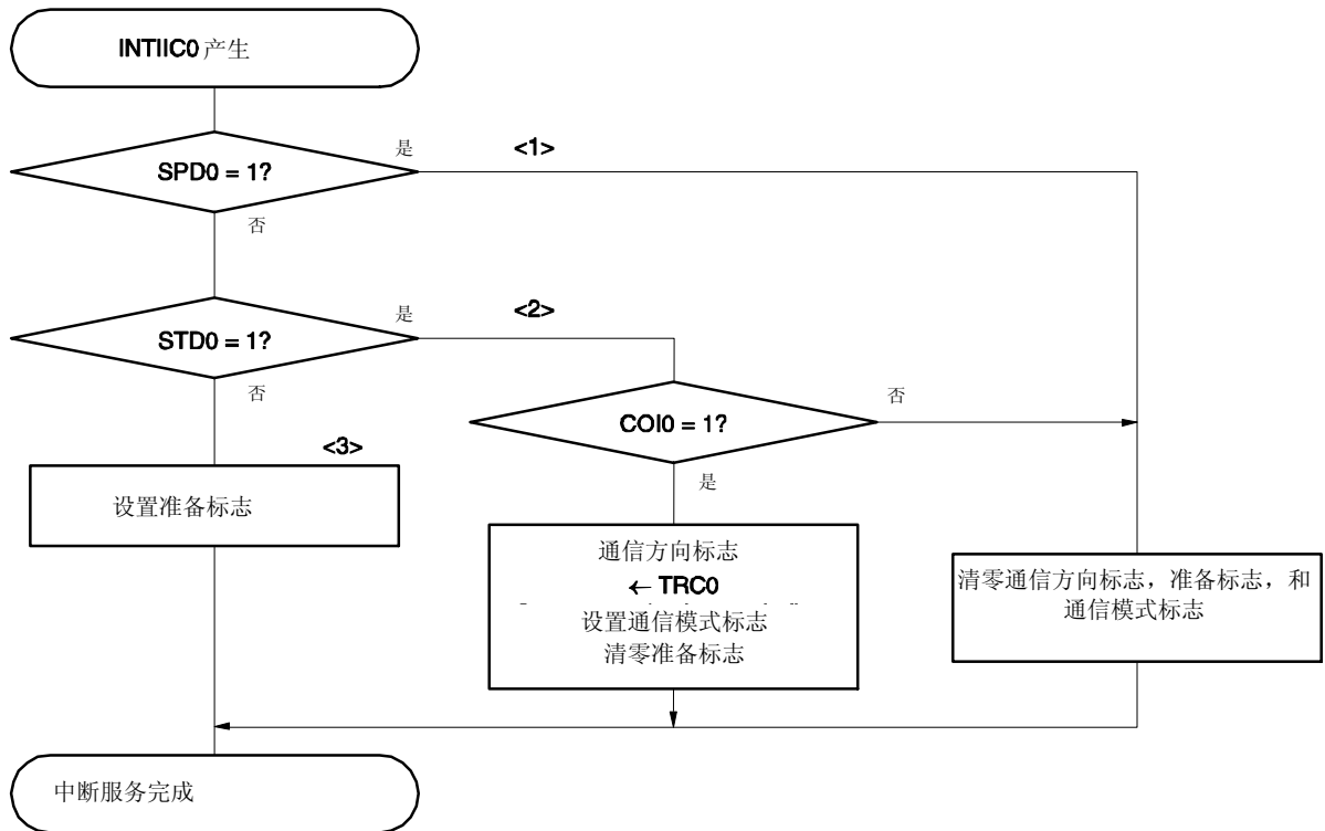
图 18-26. 从设备操作流程图中(2)
