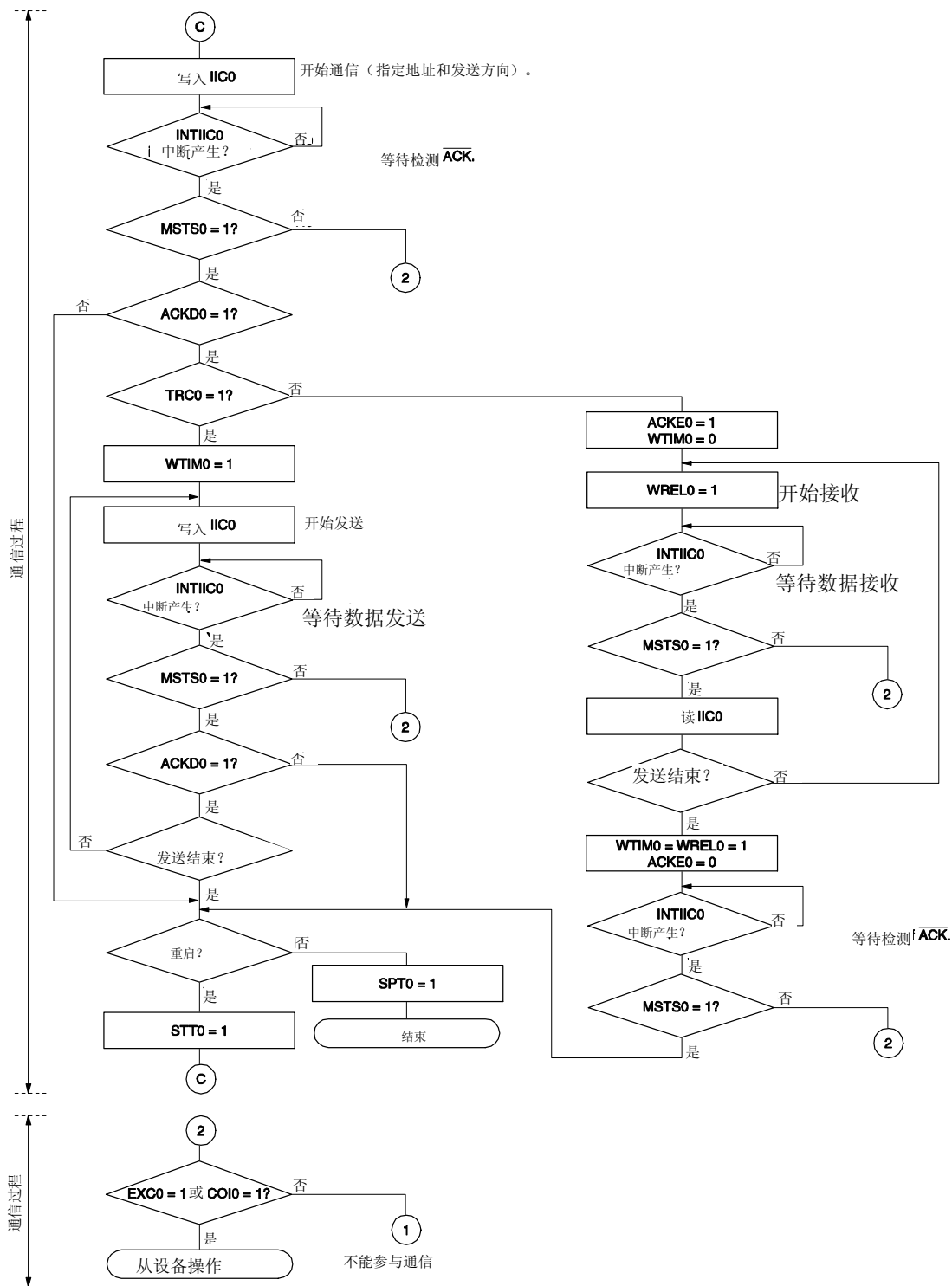
图 18-24. 主设备操作(多主设备系统) (3/3)
