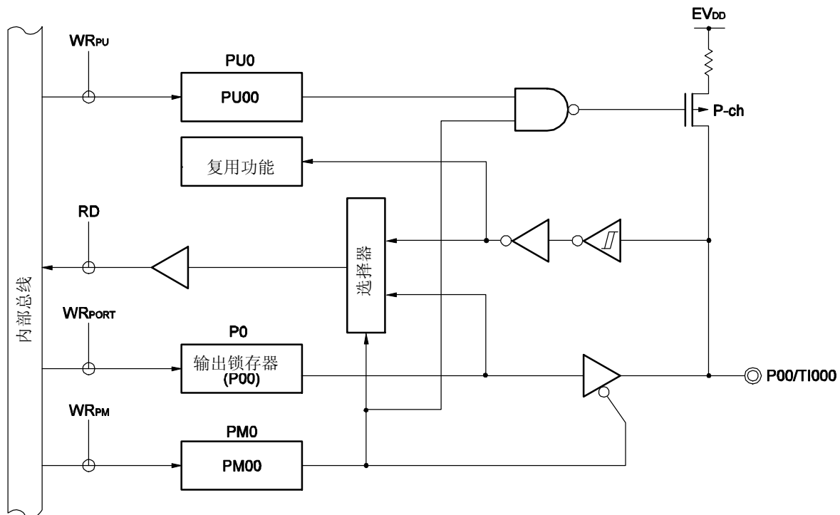
图 5-1. P00 的框图
