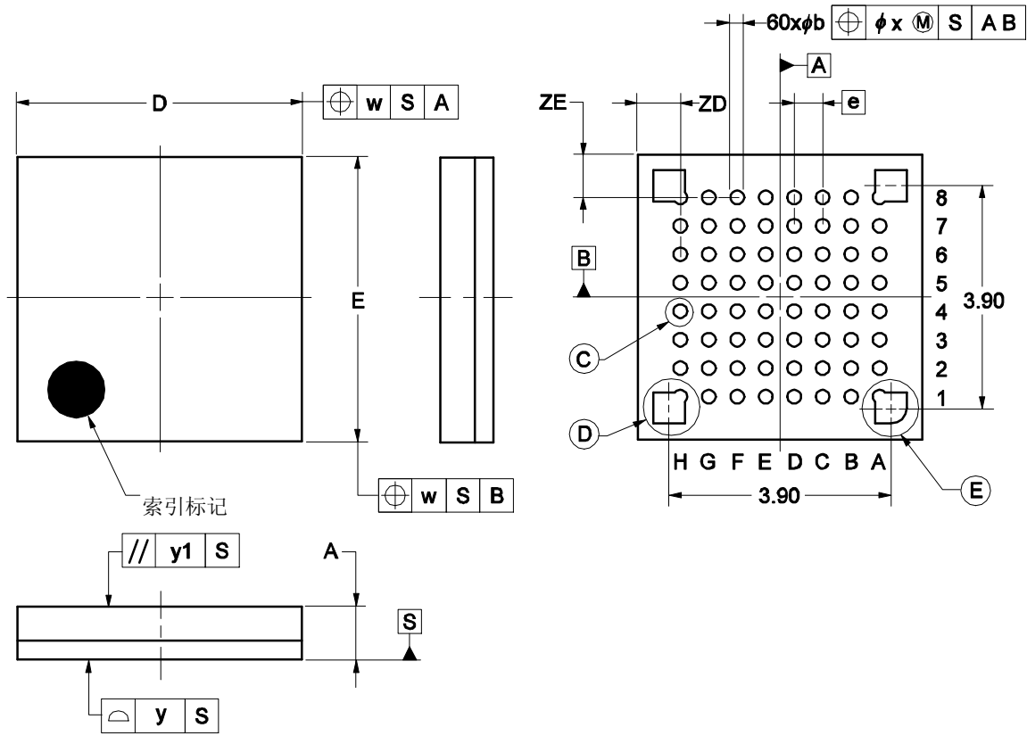
© 部分详端图
