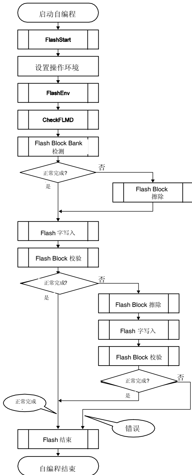
图 27-14. 自编程的流程(重写 Flash 存储器)
