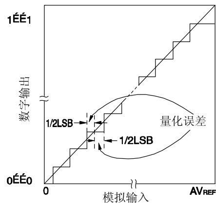
图 13-15. 量化误差
