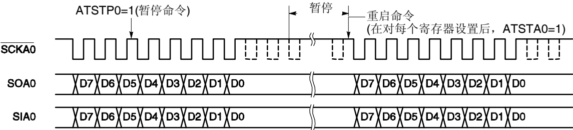
图 17-22 自动发送/接收操作的暂停和重新启动
