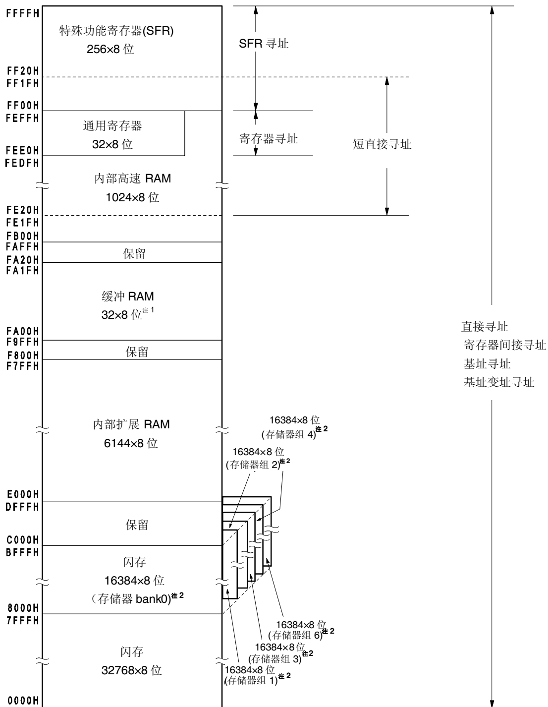
图 3-19. 数据存储空间与寻址方式的对应关系 ( \mu PD78F0527A, 78F0537A, 78F0547A, 78F0527DA, 78F0537DA, 78F0547DA)
