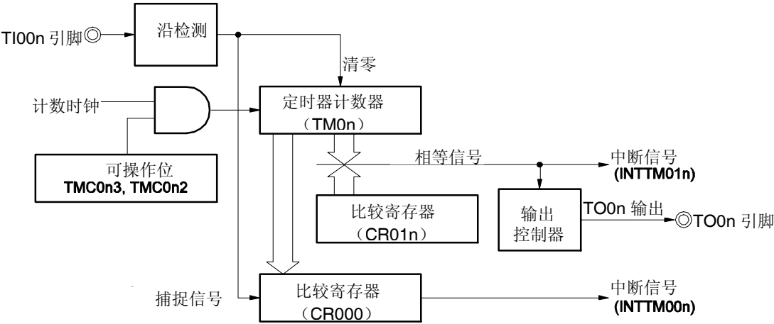
图 7-31 清零&启动模式(通过 TI00n 引脚有效沿输入进入)的框图 (CR00n: 捕捉寄存器, CR01n: 比较寄存器)
