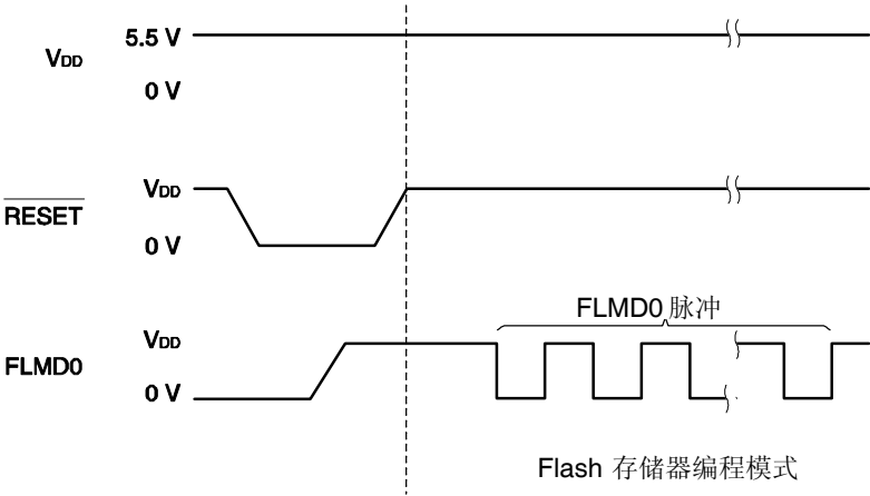
图 27-11. Flash 存储器编程模式
