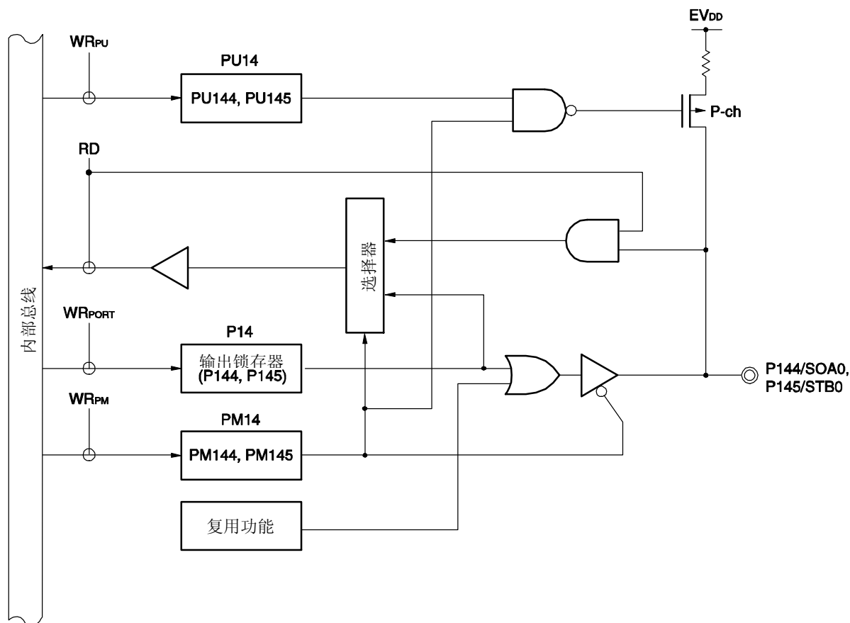
图 5-28. P144 和 P145 的框图
