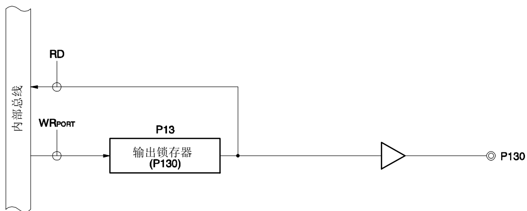
图 5-24. P130 的框图
