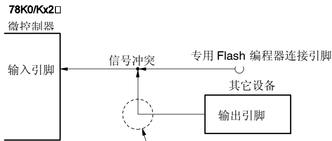
图 27-7. 信号冲突 (串行接口的输入引脚)
