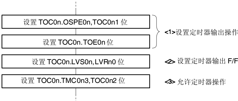
图 7-58 LVS0n 和 LVR0n 设置流程示例
