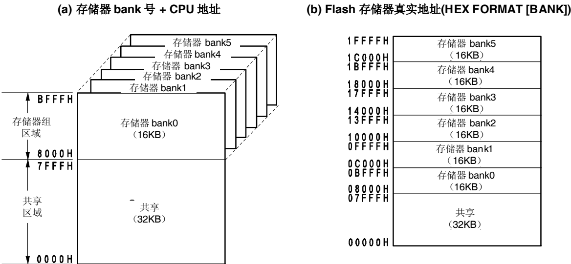
图 4-2. 地址示意图
