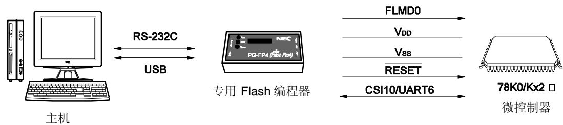
图 27-3. Flash 存储器编程环境
