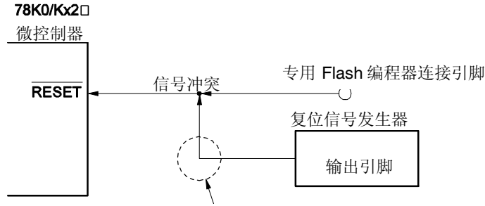
图 27-9. 信号冲突 (RESET 引脚)
