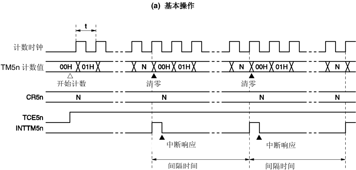
图 8-11. 间隔定时器操作的时序(1/2)
