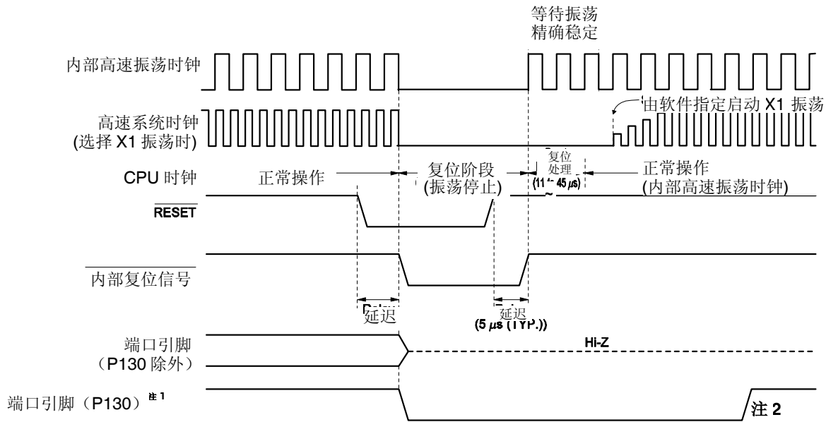
图 23-2. 由 RESET 输入进行复位的时序
