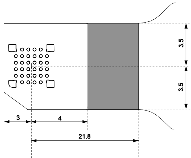
图 B-2. 对于 36 引脚 FC 封装
