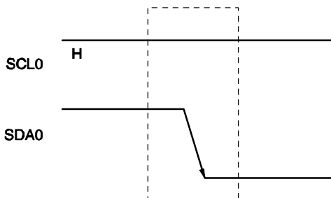
图 18-13. 起始条件
