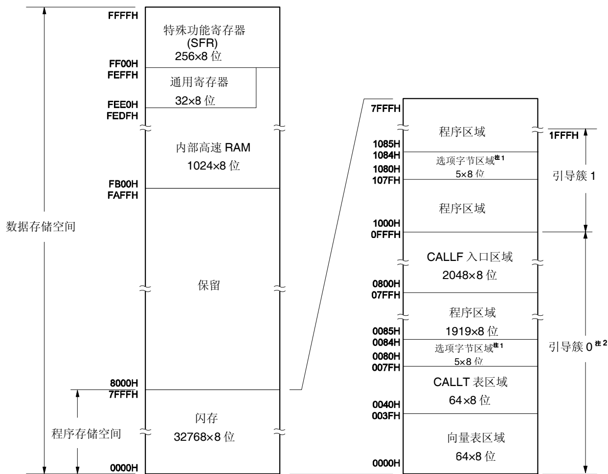
图 3-4. 存储空间映射图 (μPD78F0503A, 78F0513A, 78F0523A, 78F0533A)
