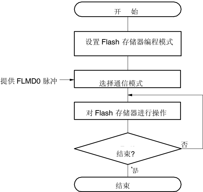
图 27-10. Flash 存储器操作过程
