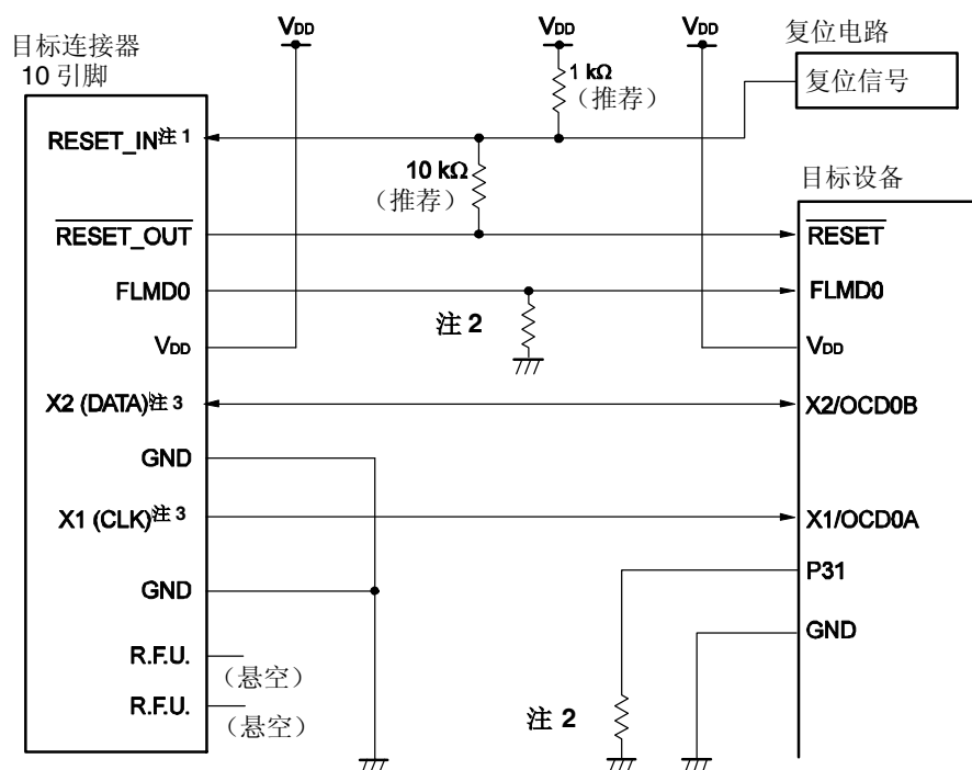
图 28-1. QB-78K0MINI 或 QB-MINI2 和 \mu PD78F05xxDA 的连接示例 (当使用 OCD0A/X1 和 OCD0B/X2 时)
