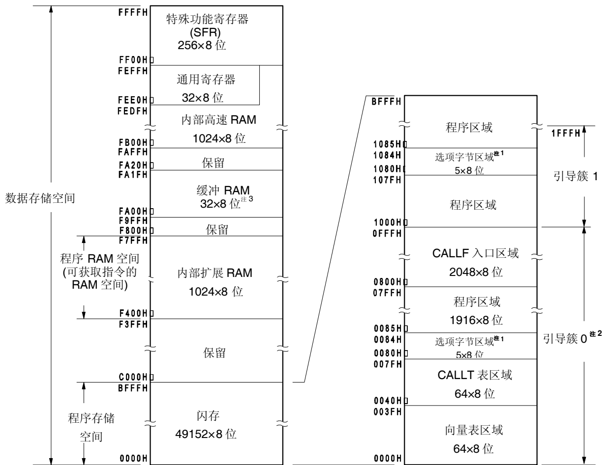
图 3-6. 存储空间映射图 (μPD78F0514A, 78F0524A, 78F0534A, 78F0544A)
