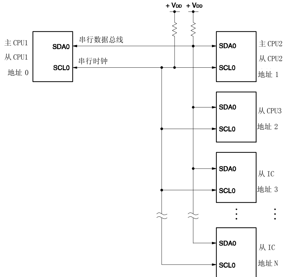
图 18-2. 使用 I 2 C 总线的串行总线配置举例
