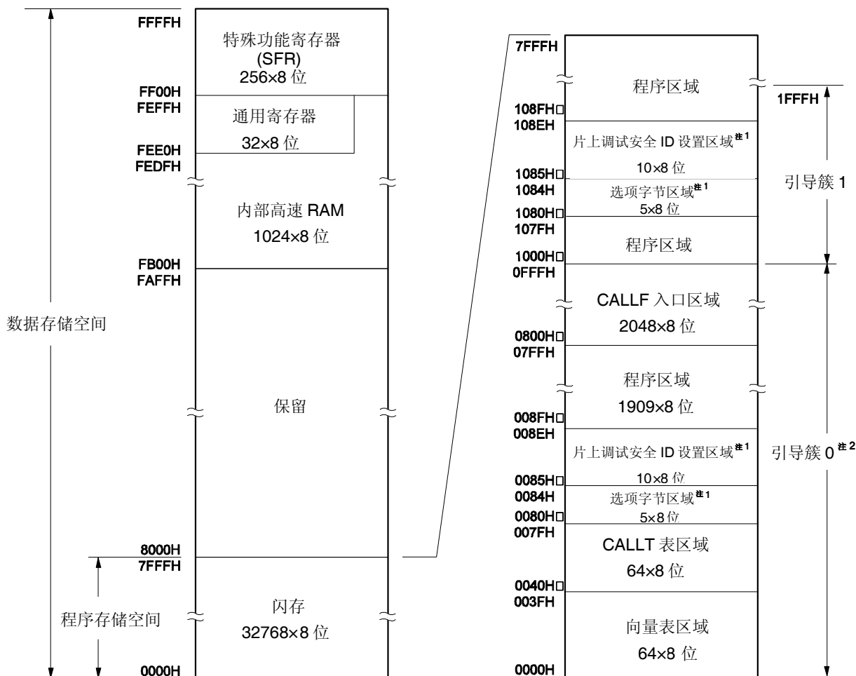
图 3-5. 存储空间映射图 (μPD78F0503DA, 78F0513DA)
