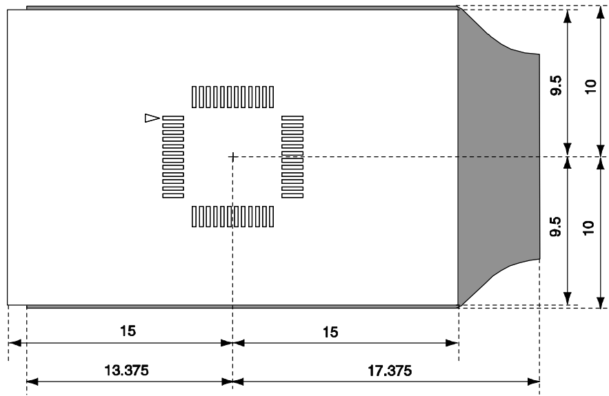
图 B-4. 对于 48 引脚 GA 封装
