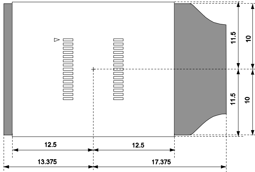
图 B-1. 对于 30 引脚 MC 封装
