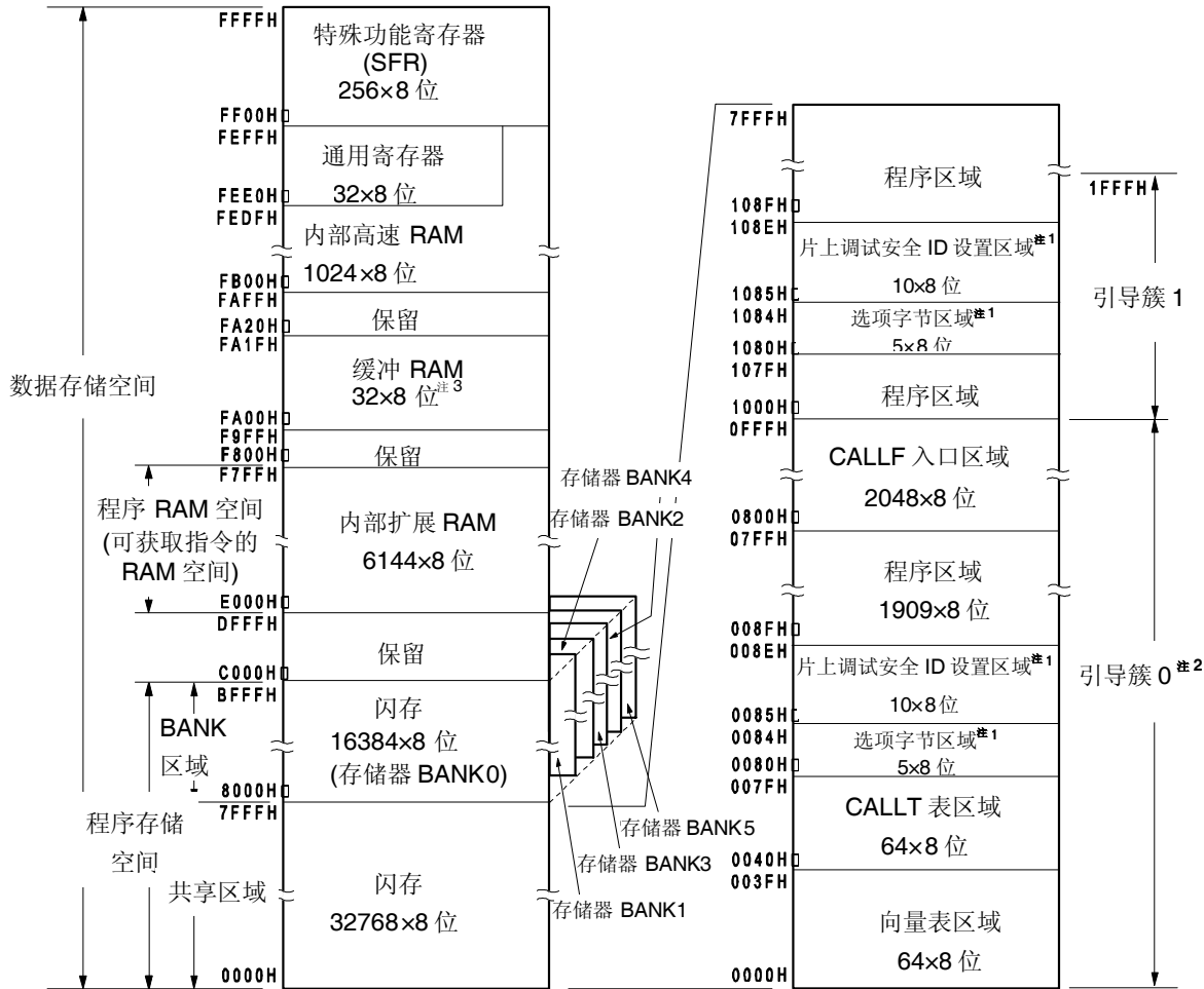
图 3-11. 存储空间映射图 (μPD78F0527DA, 78F0537DA, 78F0547DA)
