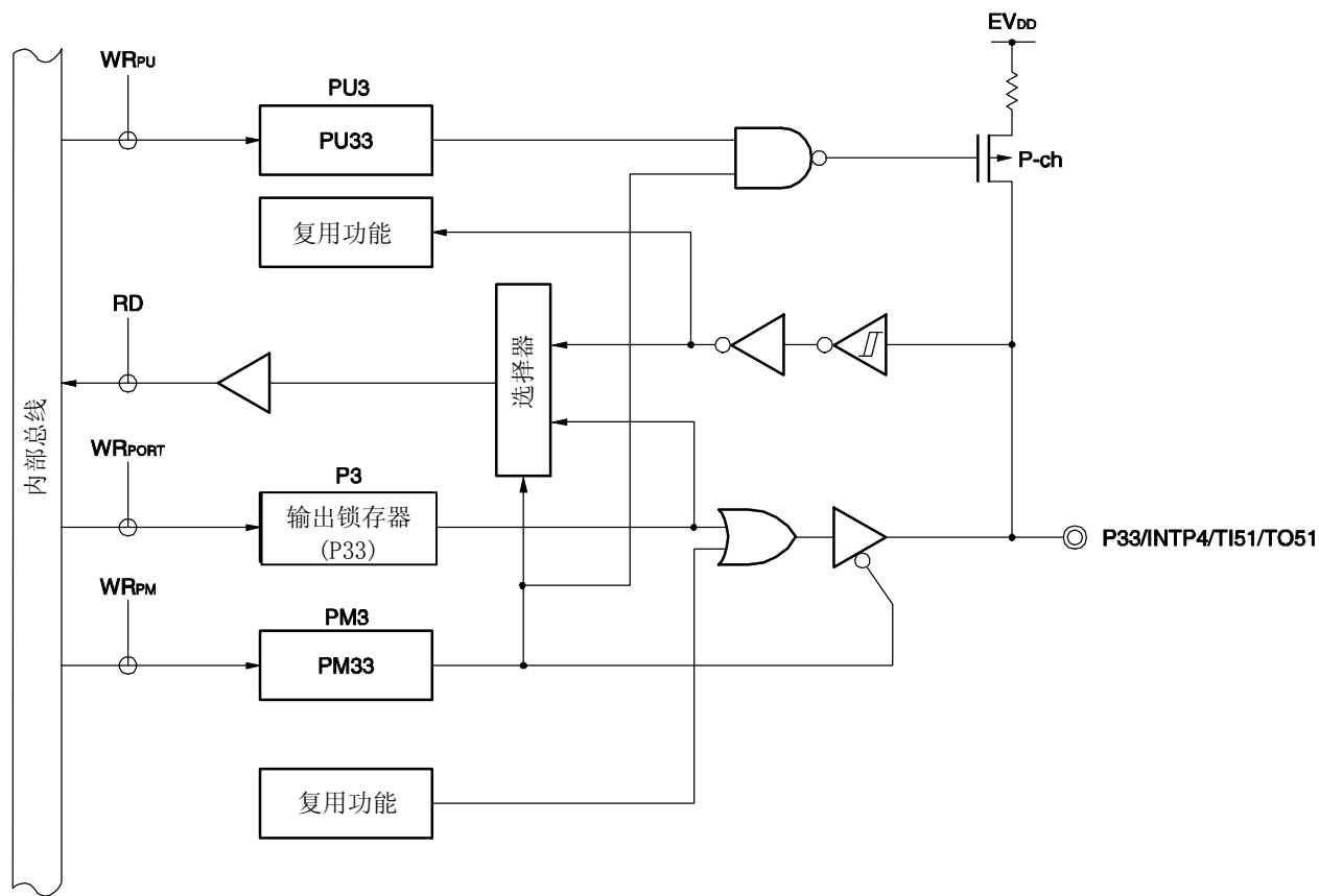
图 5-14. P33 的框图
