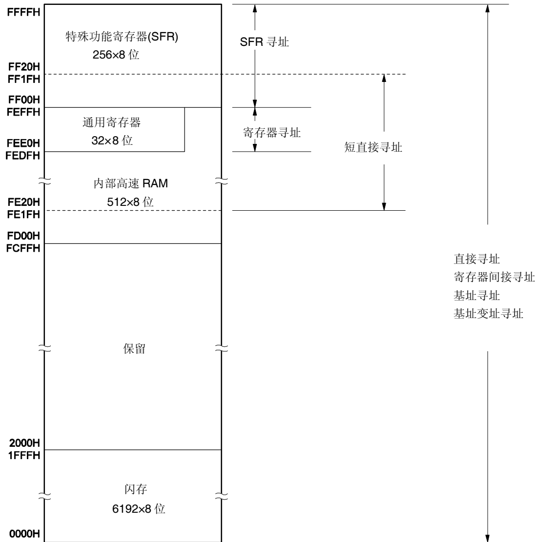
图 3-12. 数据存储空间与寻址方式的对应关系 (μPD78F0500A)
