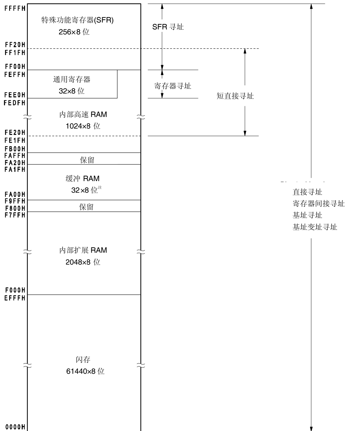
图 3-17. 数据存储空间与寻址方式的对应关系 ( \mu PD78F0515A, 78F0525A, 78F0535A, 78F0545A, 78F0515DA)
