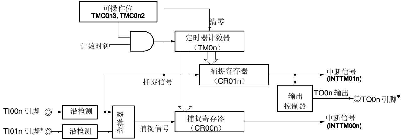
图 7-33 清零&启动模式(通过 TI00n 引脚有效沿输入进入)的框图 (CR00n: 捕捉寄存器, CR01n: 捕捉寄存器)
