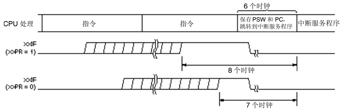
图 20-20. 中断请求响应时序(最短时间)
