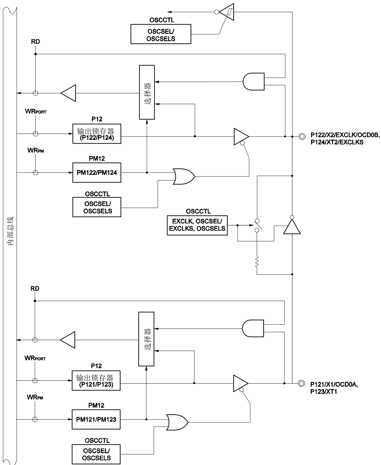
图 5-23. 的框图 P121~P124
