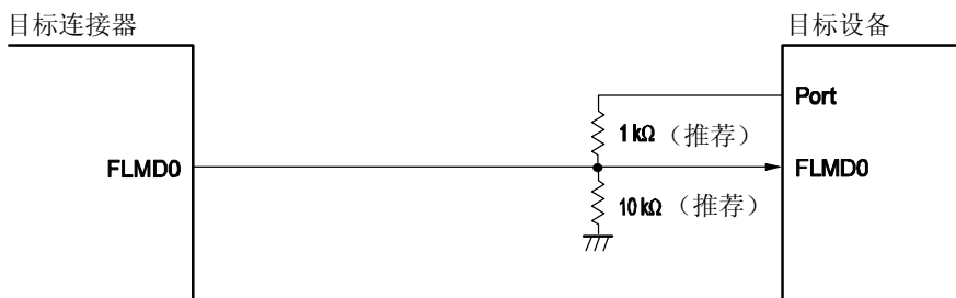
图 28-3. 通过片上调试进行自编程时的 FLMD0 引脚连接
