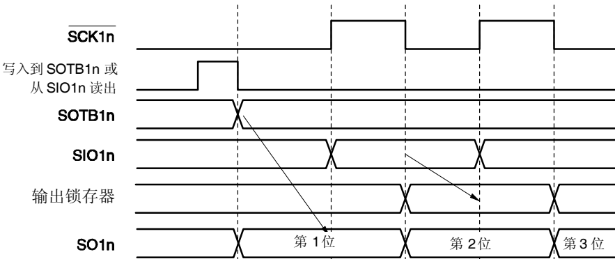
(d) 类型 4: CKP1n = 1, DAP1n = 1
