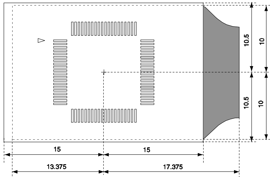
图 B-12. 对于 80 引脚 GK 封装
