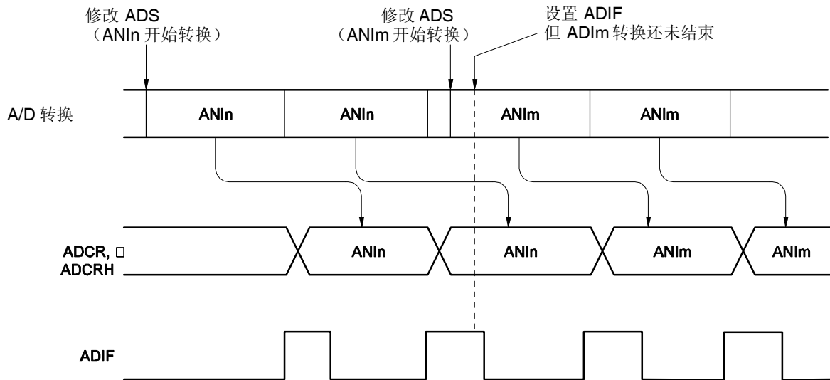
图 13-21. A/D 转换结束中断请求产生的时序
