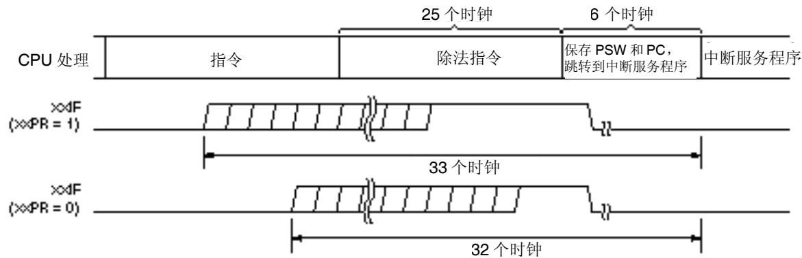
图 20-21. 中断请求响应时序(最长时间)
