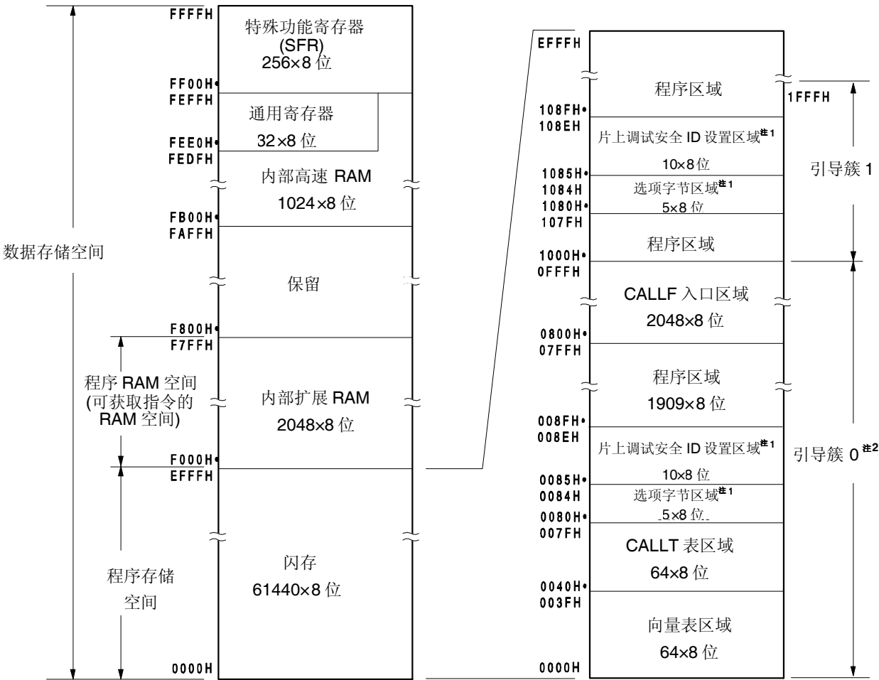
图 3-8. 存储空间映射图 (μPD78F0515DA)
