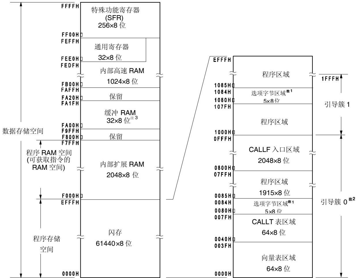
图 3-7. 存储空间映射图 (μPD78F0515A, 78F0525A, 78F0535A, 78F0545A)
