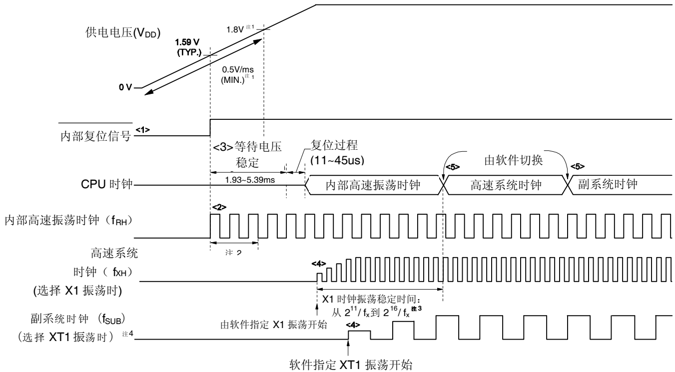
图 6-15. 上电时的时钟发生器操作 (设置 1.59 V POC 模式 (选项字节: POCMODE = 0))
