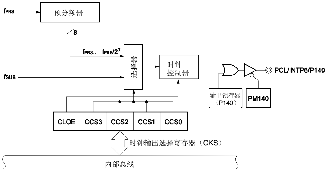
图 12-1 时钟输出/蜂鸣器输出控制器的框图(78K0/KC2 系列 48 引脚产品, 78K0/KD2)
