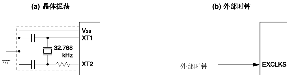
图 6-13. XT1 振荡器的外部电路示例
