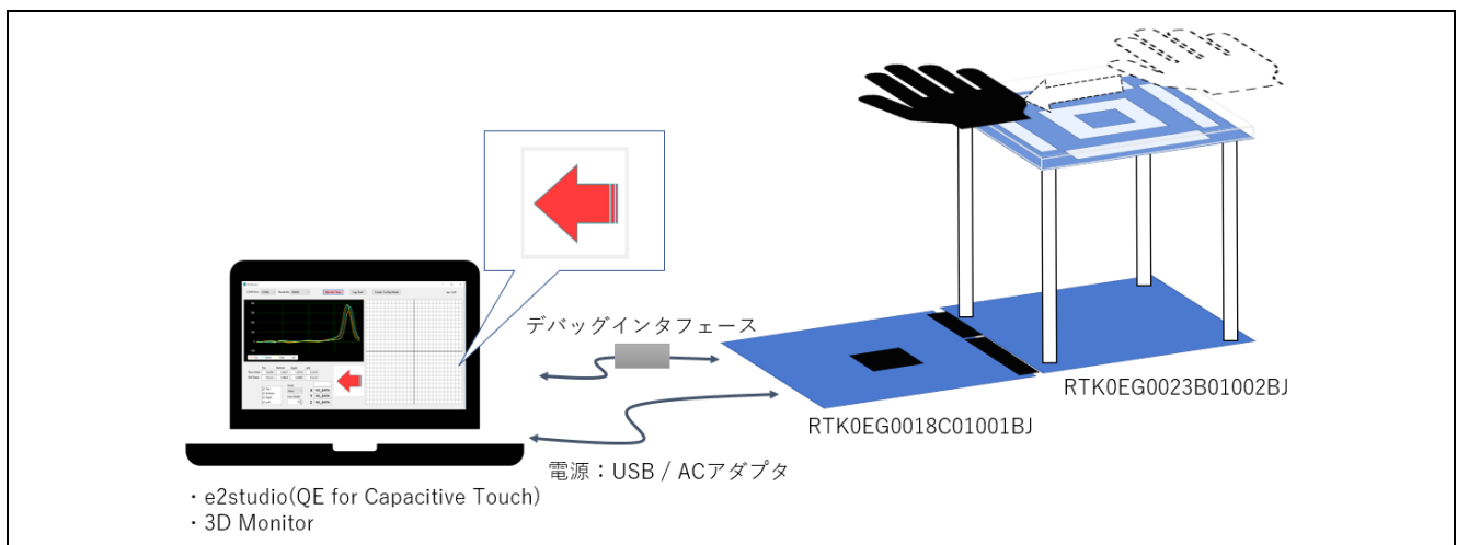
図 1-1 3D ジェスチャ電極ボード システム
