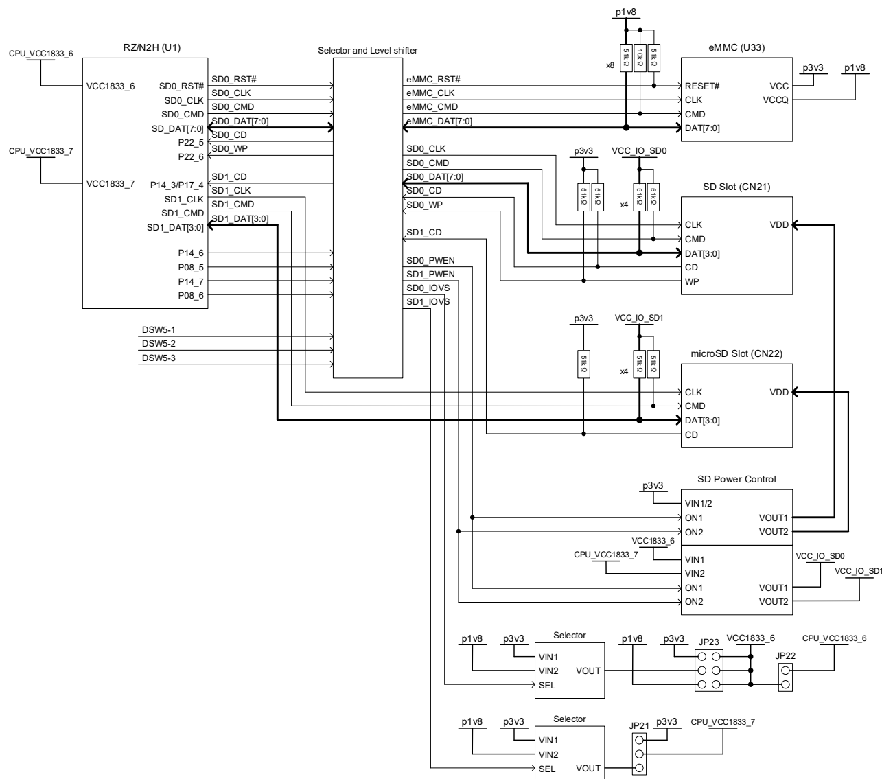
図 7-18 SD, eMMC 回路構成
