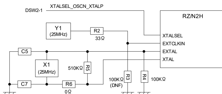
図 7-2 クロック回路
