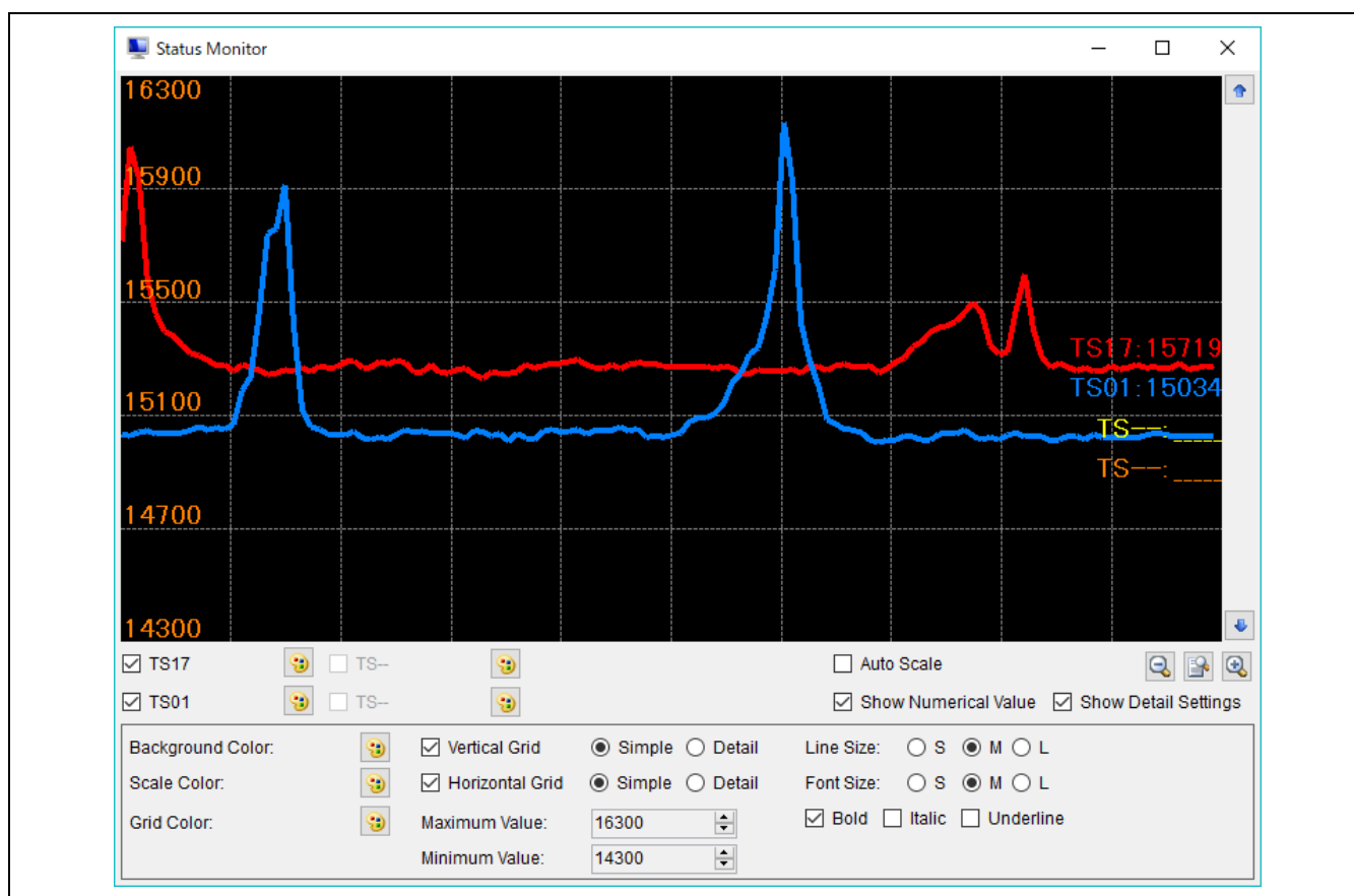
図 3.1 Status Monitor
