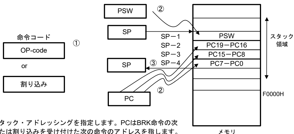
図3-45 割り込み、BRKの例
