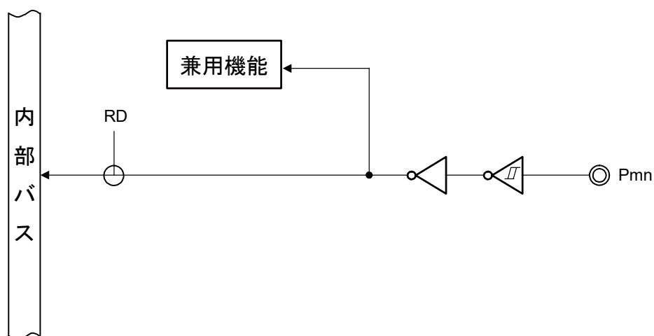
図2-3 端子タイプ 2-1-2 の端子ブロック図
