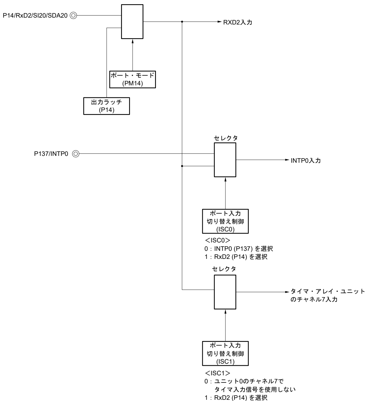
図12-102 LINの受信操作作用のポート構成図 (30, 32, 36, 40ピン製品の場合)
