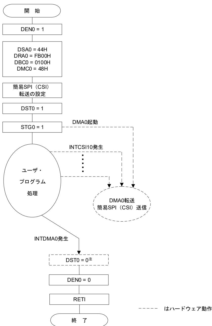
図15-7 簡易SPI (CSI) I連続送信の設定例
