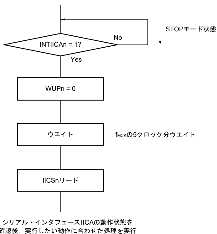
図13-23 アドレス一致によりWUPn = 0に設定する場合のフロー（拡張コード受信含む）
