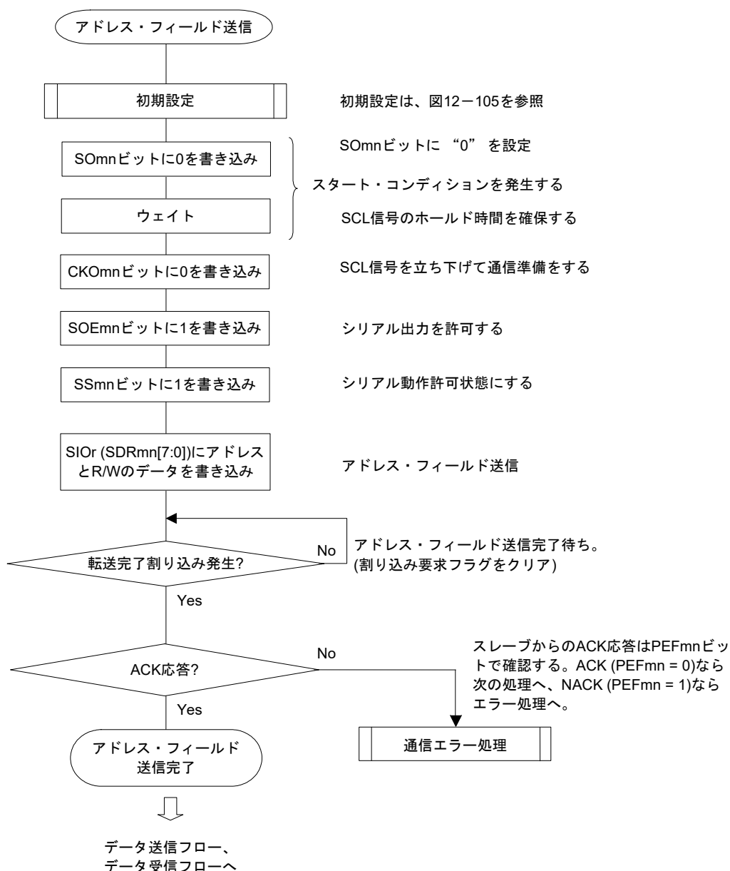
図12-107 簡易I 2 Cアドレス・フィールド送信のフロー・チャート
