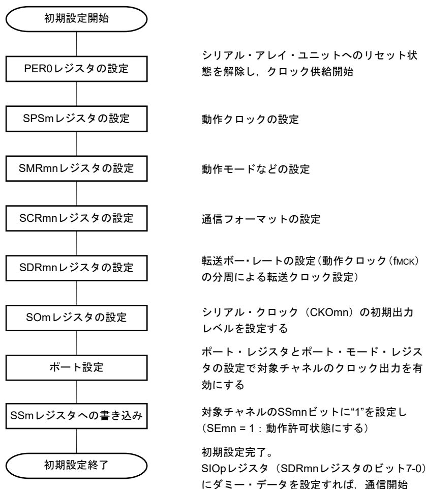
図12-34 マスタ受信の初期設定手順
