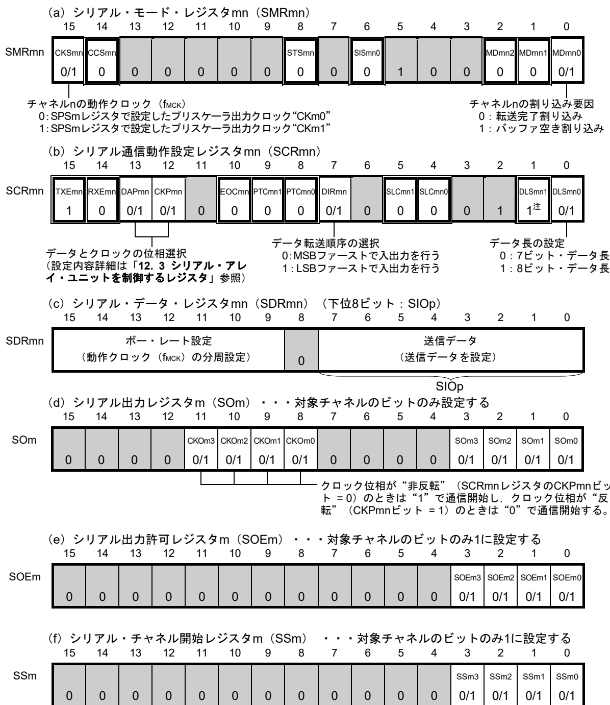
図12-25 簡易SPI (CSI00, CSI01, CSI10, CSI11, CSI20, CSI21, CSI30, CSI31) の マスタ送信時のレジスタ設定内容例
