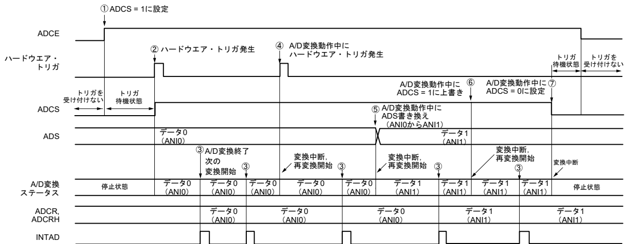
図11-25 ハードウェア・トリガ・ウェイト・モード（セレクト・モード，連続変換モード） 動作タイミング例
