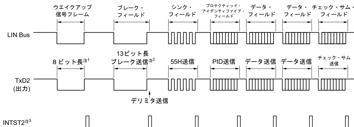
図12-98 LINの送信操作
