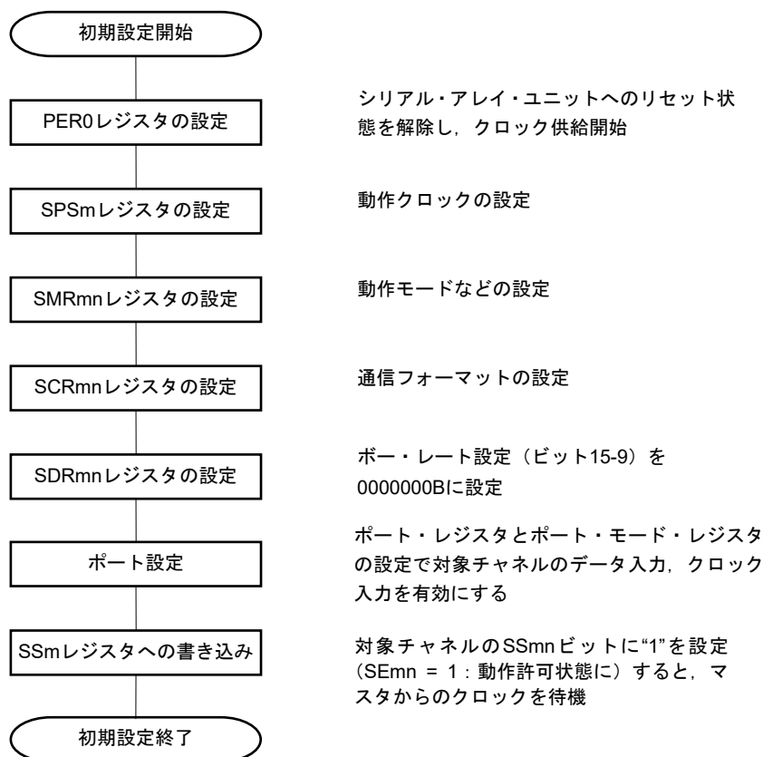
図12-58 スレーブ受信の初期設定手順
