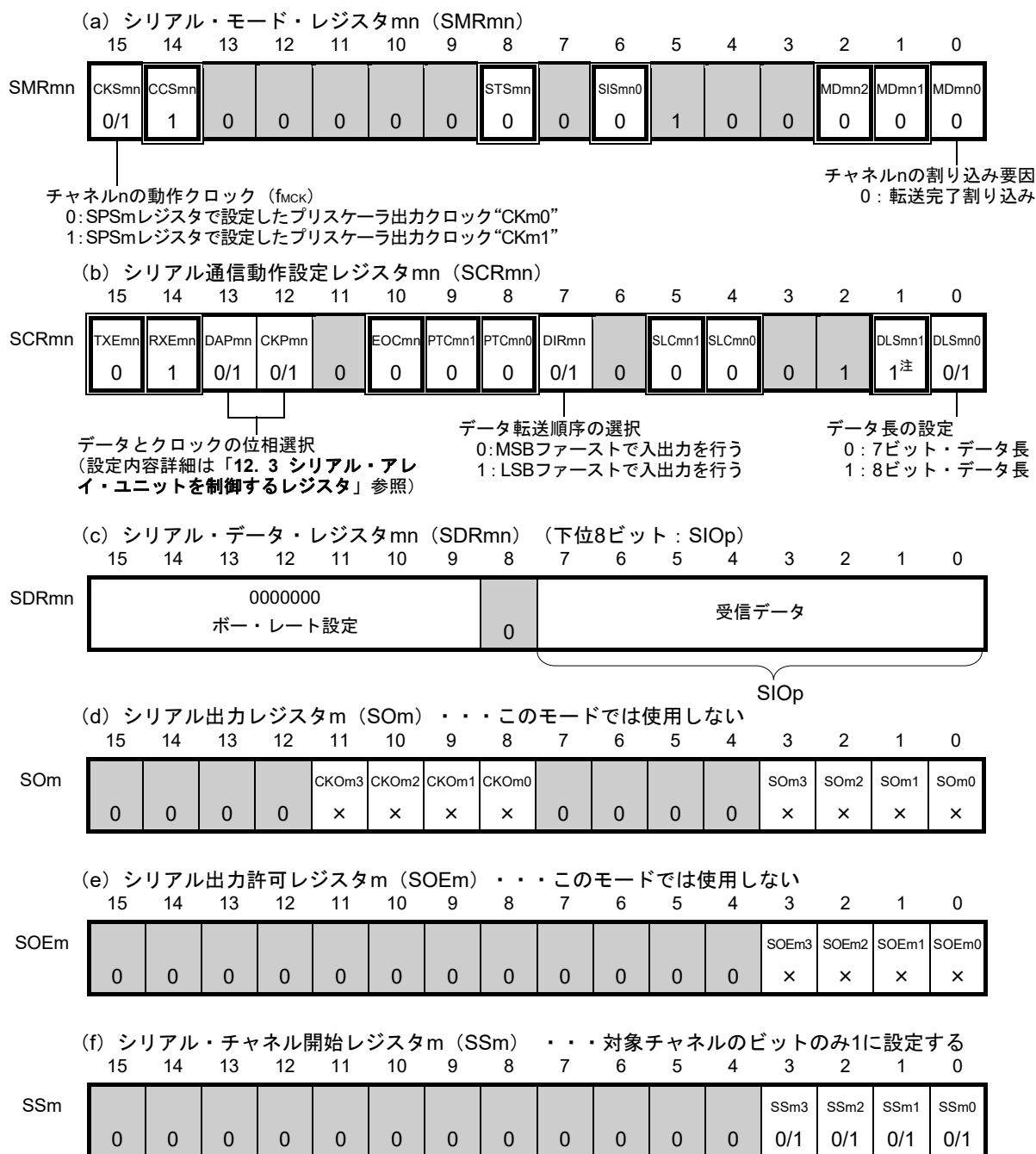
図12-57 簡易SPI (CSI00, CSI01, CSI10, CSI11, CSI20, CSI21, CSI30, CSI31) のスレーブ受信時のレジスタ設定内容例
