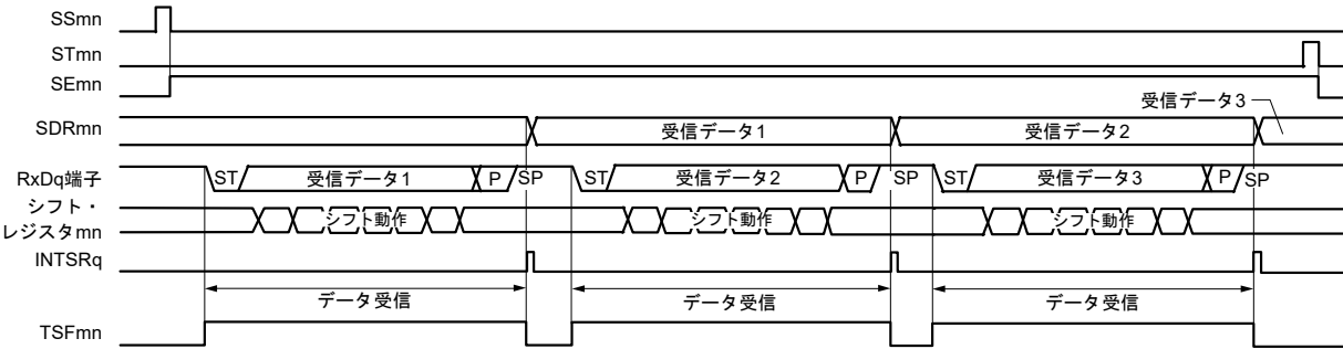
図12-88 UART受信のタイミング・チャート
