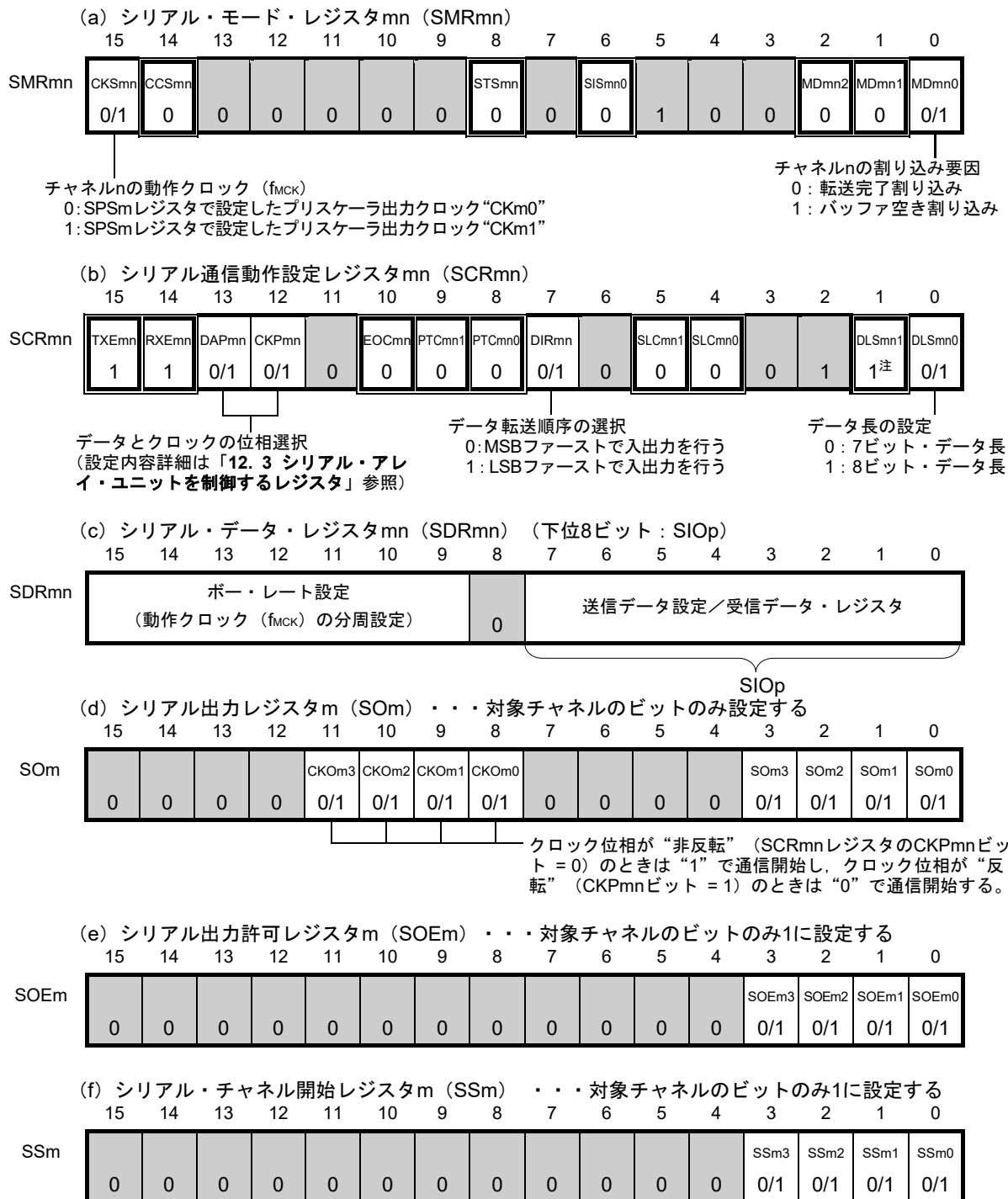
図12-41 簡易SPI (CSI00, CSI01, CSI10, CSI11, CSI20, CSI21, CSI30, CSI31) のマスタ送受信時の
