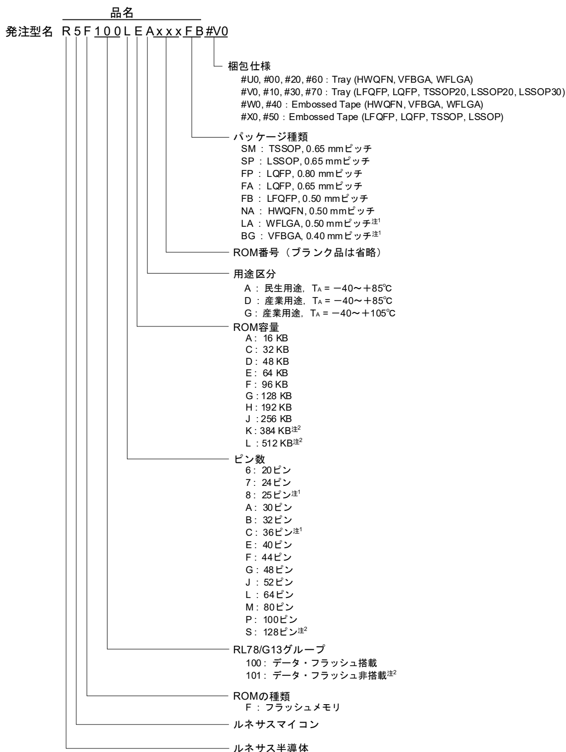
図1-1 RL78/G13の型名とメモリ・サイズ、パッケージ
