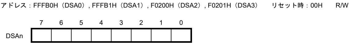
図15－1 DMA SFRアドレス・レジスタn (DSAn) のフォーマット
