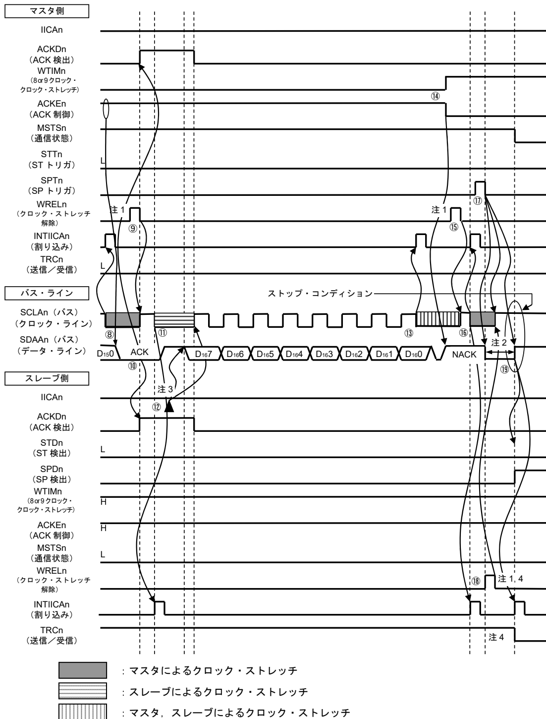
図13-33 スレーブ→マスタ通信例（マスタ：8→9クロック、スレーブ：9クロックでクロック・ストレッチ選択） (3/3)
