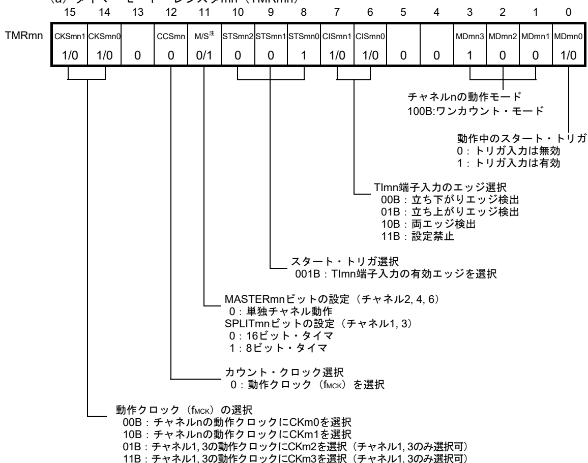
図6-63 ディレイ・カウンタ機能時のレジスタ設定内容例
