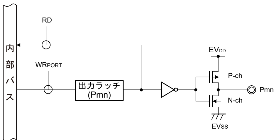
図2-2 端子タイプ 2-1-1 の端子ブロック図
