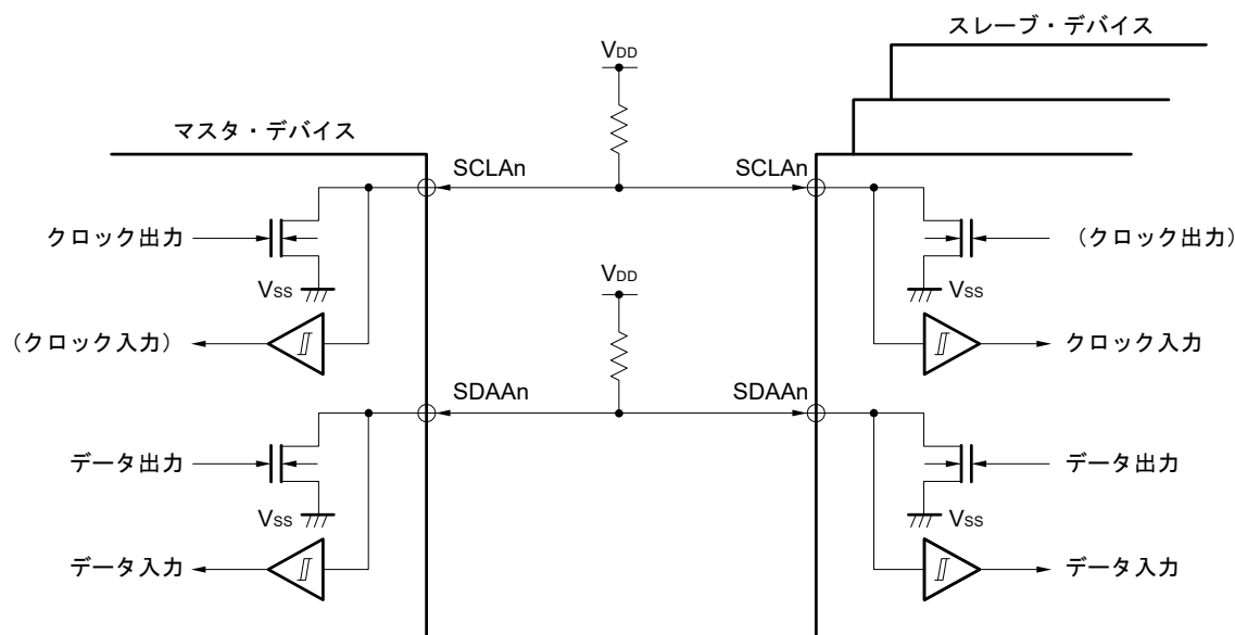
図13-13 端子構成図
