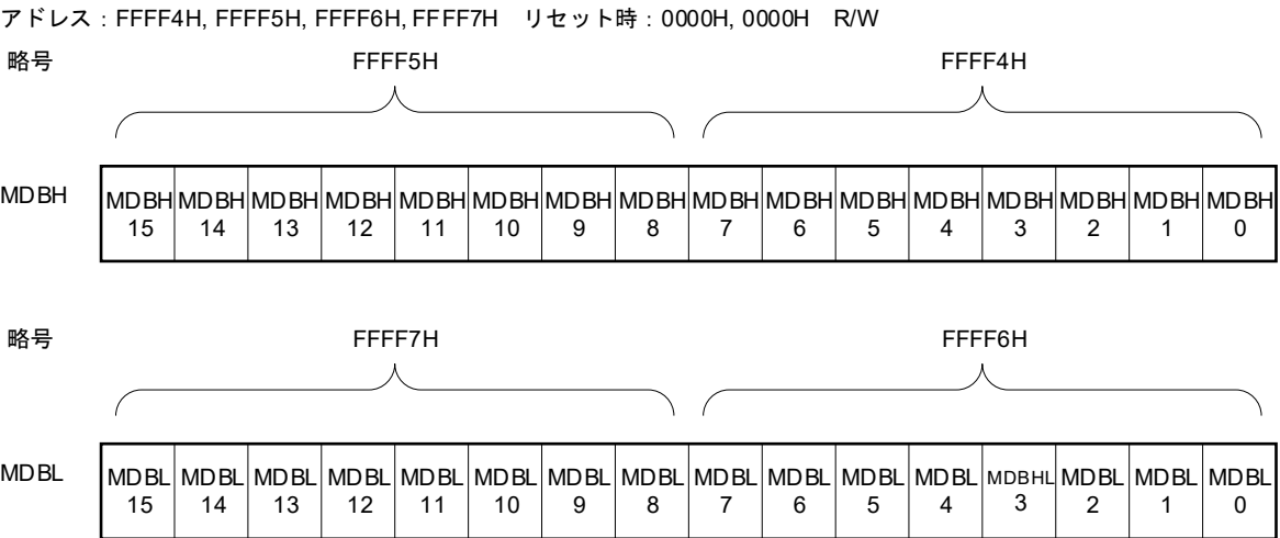
図14-3 乗除算データ・レジスタB（MDBH, MDBL）のフォーマット
