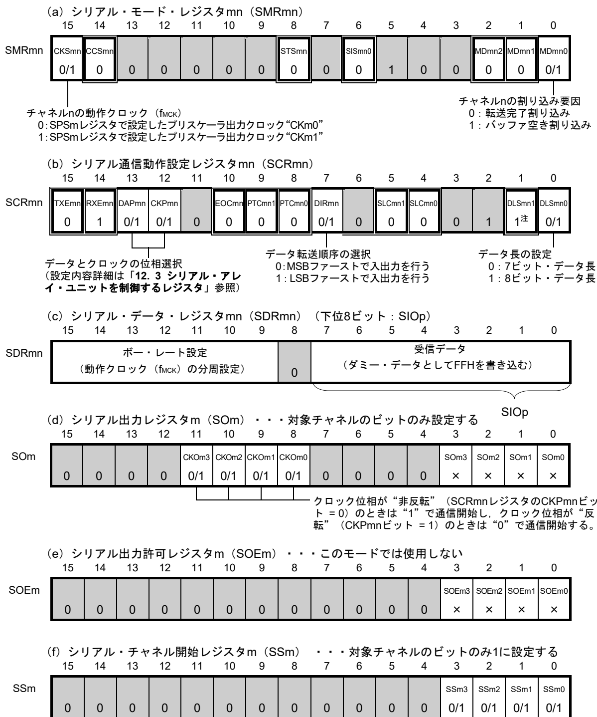
図12-33 簡易SPI (CSI00, CSI01, CSI10, CSI11, CSI20, CSI21, CSI30, CSI31) のマスタ受信時の レジスタ設定内容例
