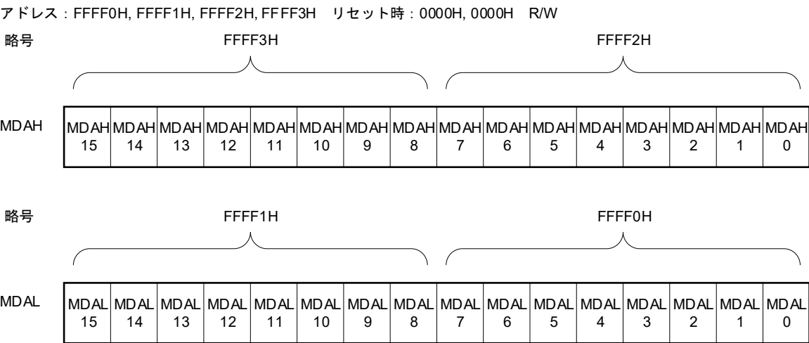
図14-2 乗除算データ・レジスタA (MDAH, MDAL) のフォーマット
