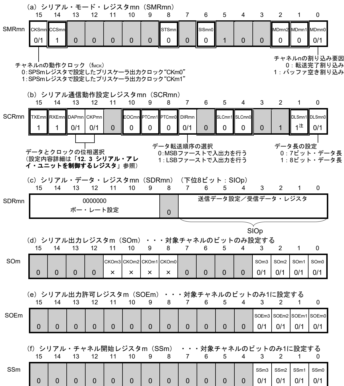
図12-63 簡易SPI (CSI00, CSI01, CSI10, CSI11, CSI20, CSI21, CSI30, CSI31) のスレーブ送受信時の レジスタ設定内容例
