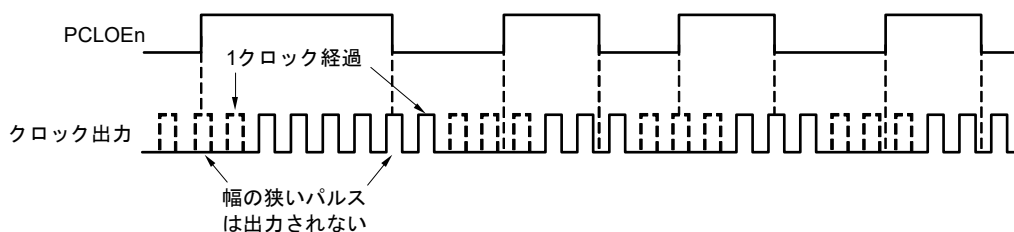
図9-3 PCLBUZn端子からのクロック出力のタイミング
