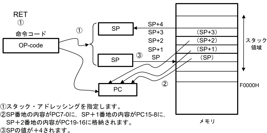
図3-44 RETの例
