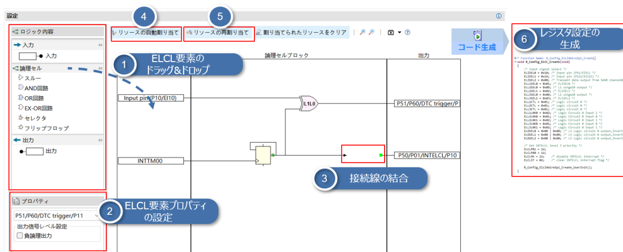
図 4-35 ELCL Flexible Circuit 作成手順
