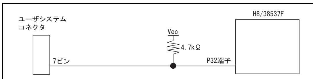
図 4.3 E8/E8a エミュレータと P32 端子の接続 (H8/38537F)
