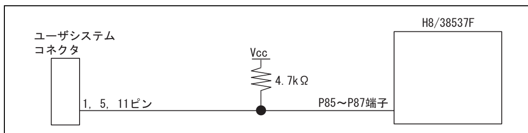
図 4.2 E8/E8a エミュレータと P85～P87 端子の接続 (H8/38537F)
