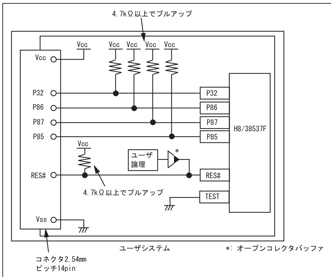
図 4.1 E8/E8a エミュレータの接続例 (H8/38537F)
