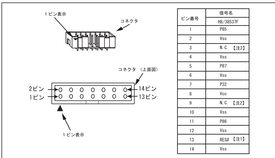
図 3.1 E8/E8a エミュレータ接続コネクタのピン配置
