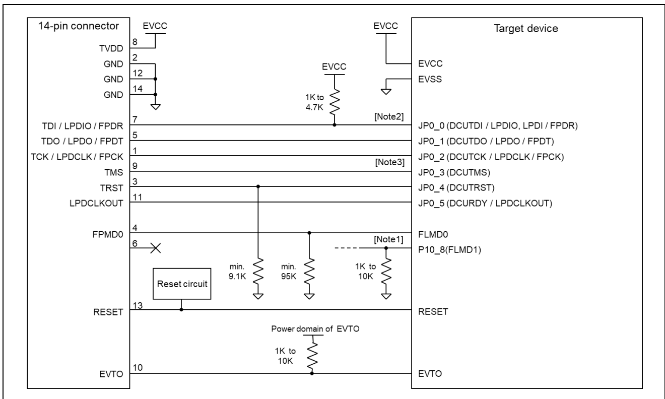
図 2-4 接続例
