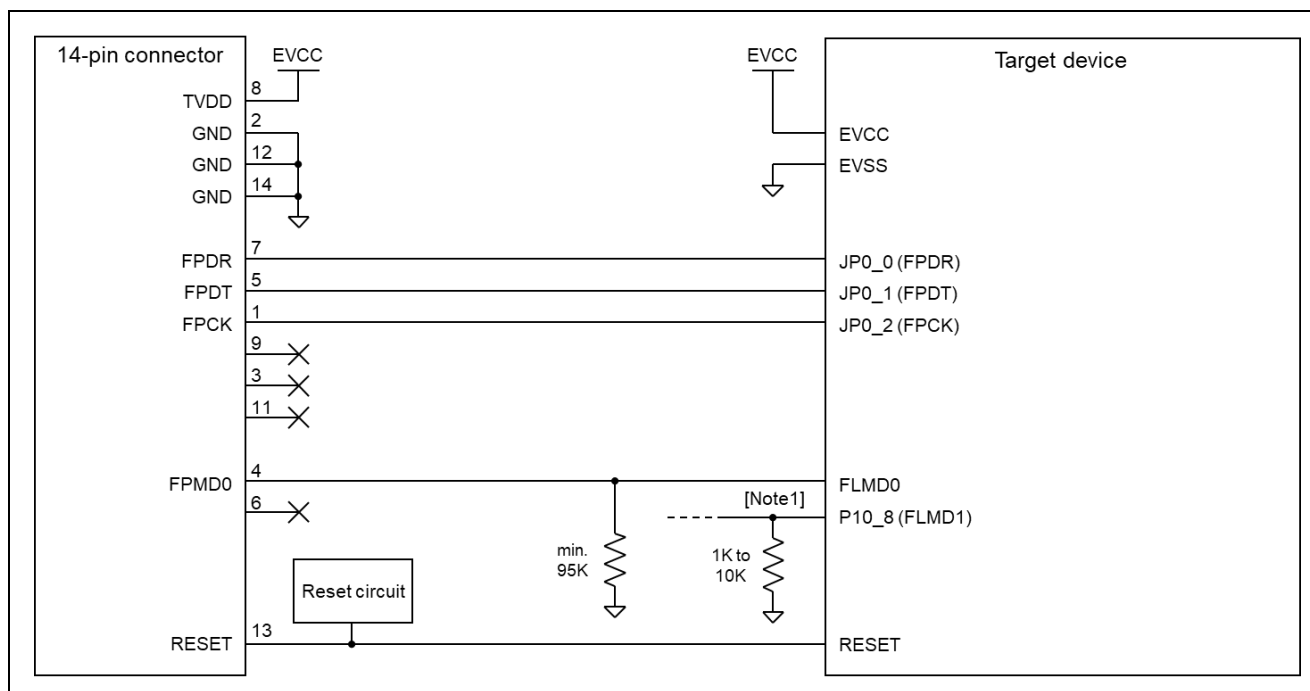
図 2-7 接続例
