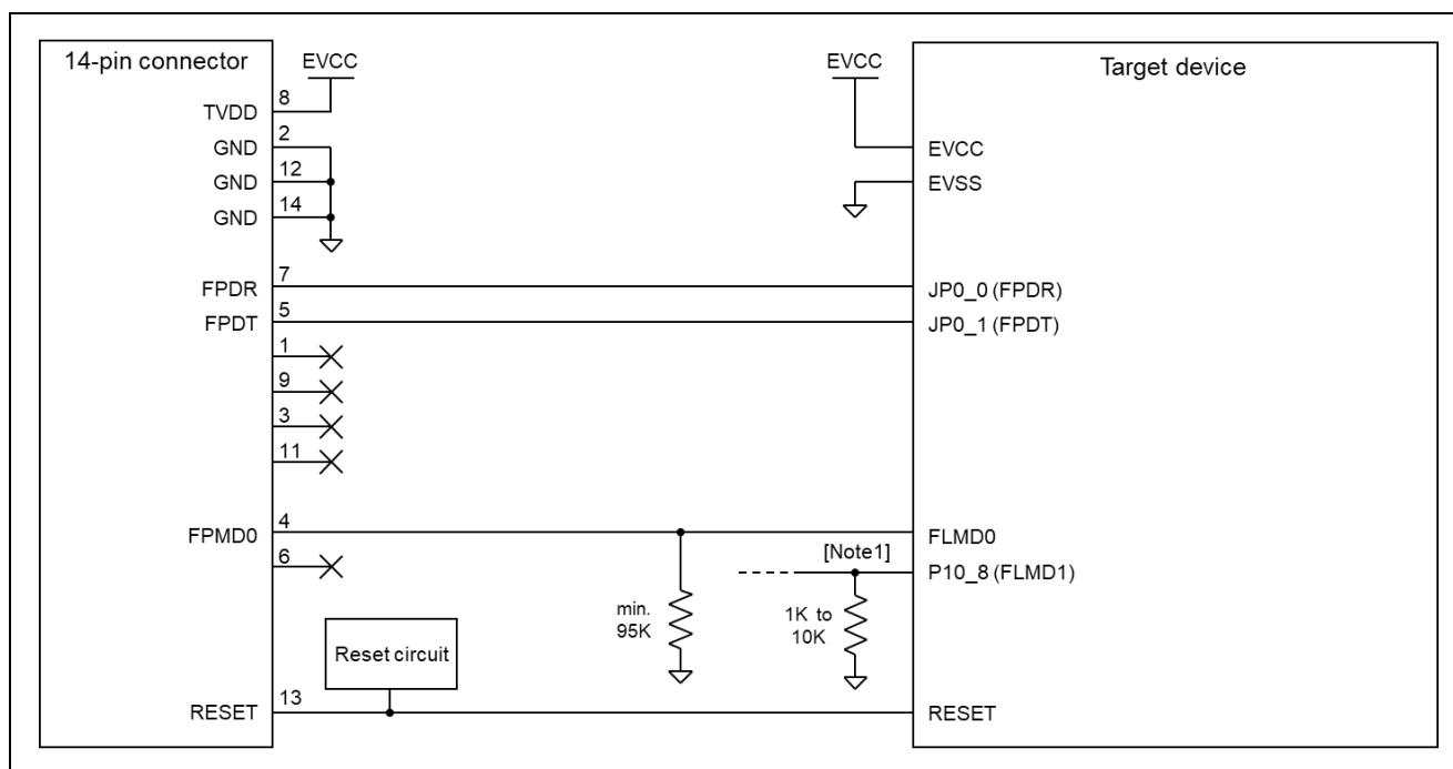
図 2-6 接続例
