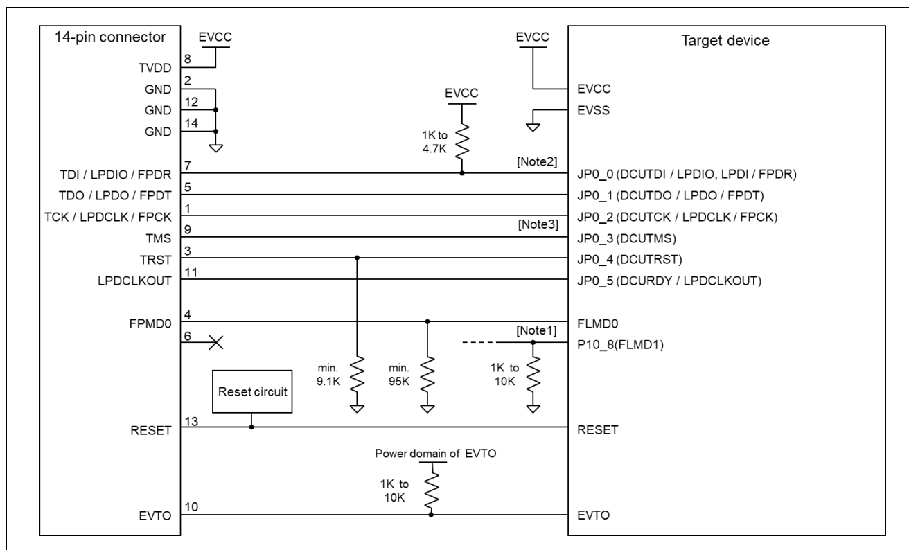
図 2-4 接続例
