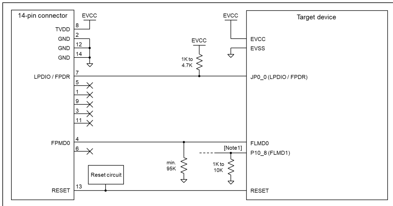
図 2-5 接続例
