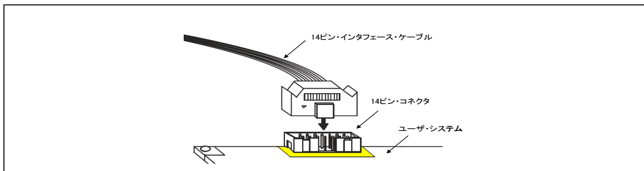
図 2-2 E1 エミュレータでの 14 ピンコネクタへのユーザインタフェースケーブル接続
