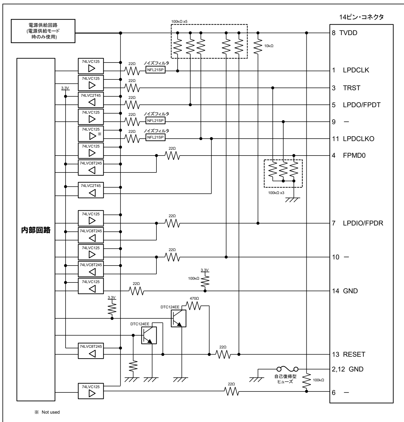
図 5-1 E1/E20 エミュレータ内インタフェース回路(LPD 4pin、2wireUART)
