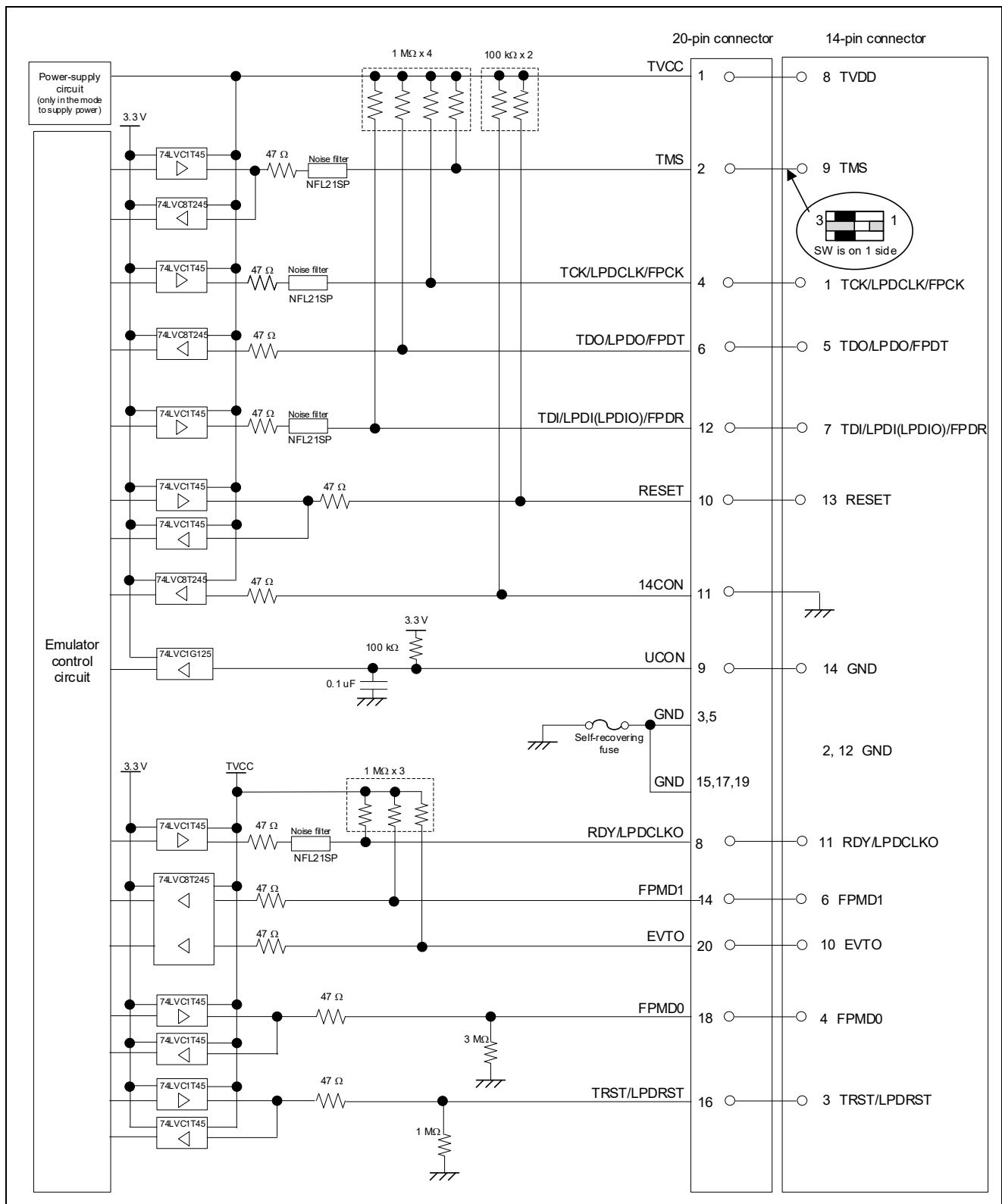
図 5-3 E2 エミュレータ (Rev.D) 内インタフェース回路 (LPD 4pin、JTAG、2wireUART、CSI)
