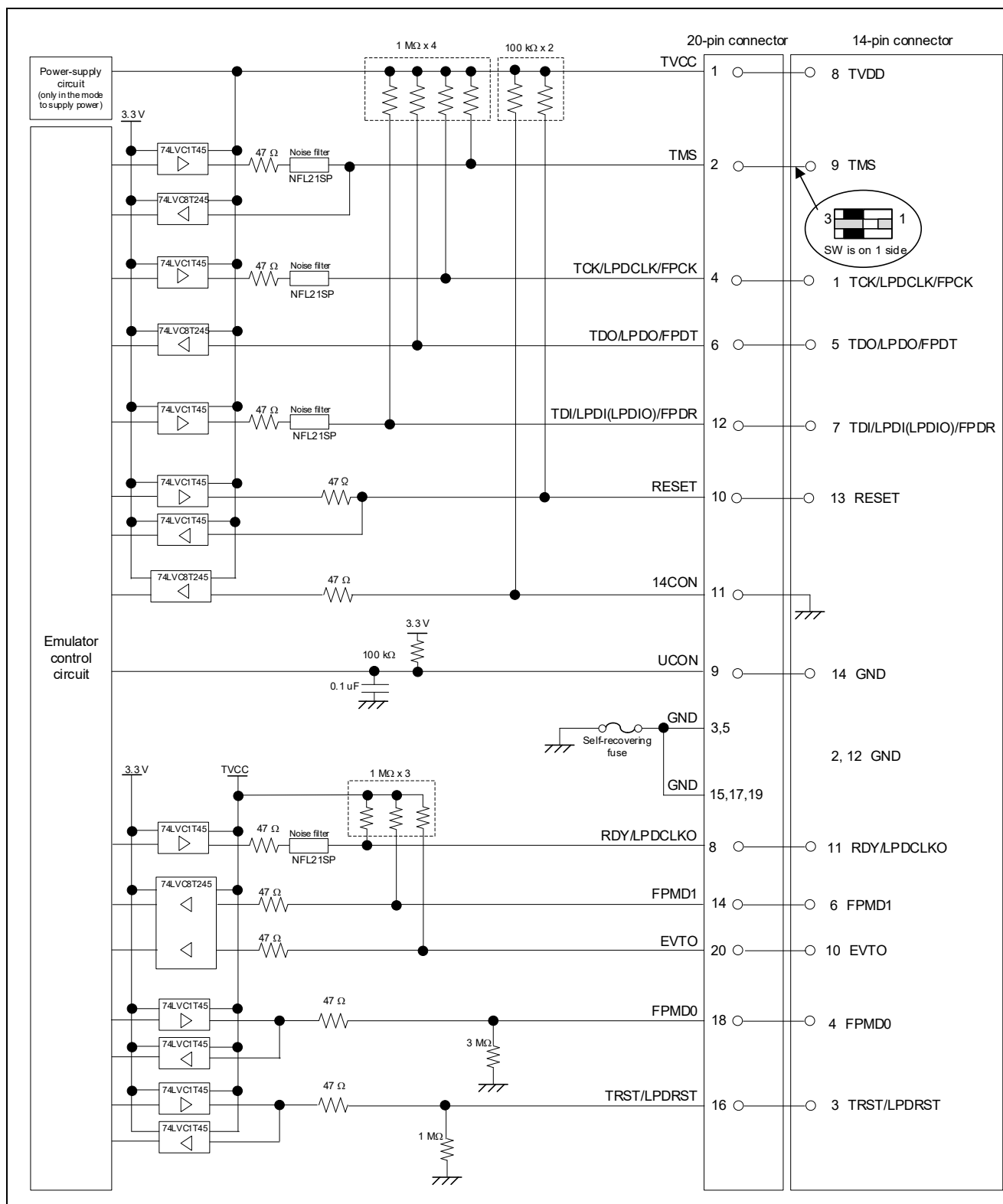
図 5-2 E2 エミュレータ (Rev.C) 内インタフェース回路 (LPD 4pin、JTAG、2wireUART、CSI)
