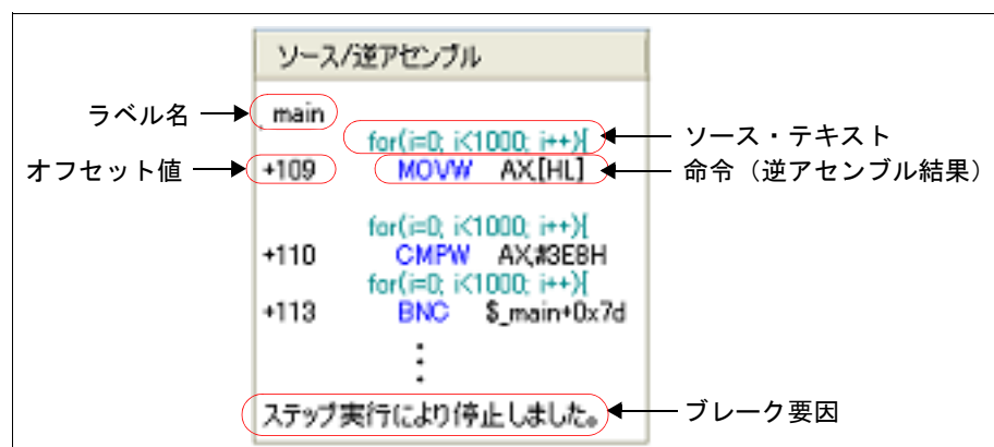
図 A.16 [ソース / 逆アセンブル] エリアの表示内容（デフォルト）
