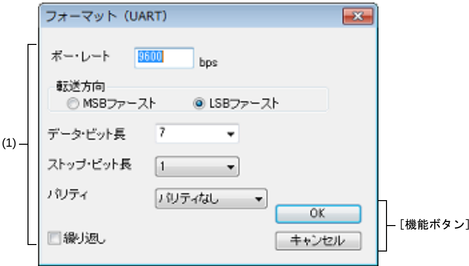
図 A.91 フォーマット（UART）ダイアログ
