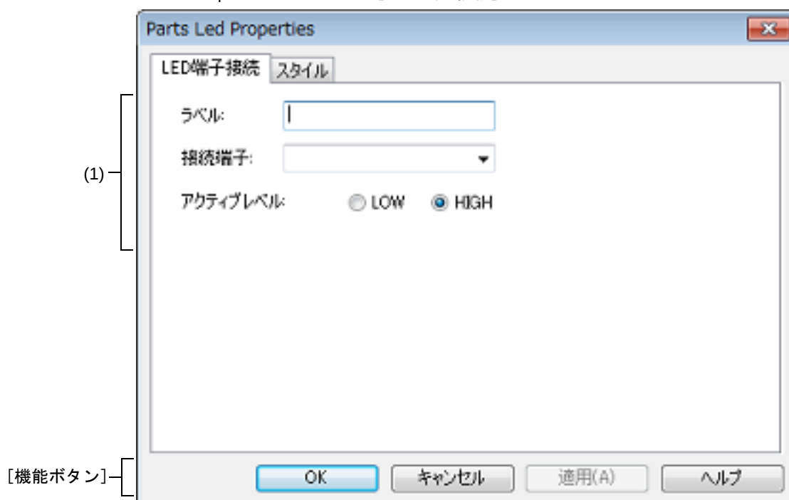
図 A.74 Parts Led Properties ダイアログ : [LED 端子接続] タブ
