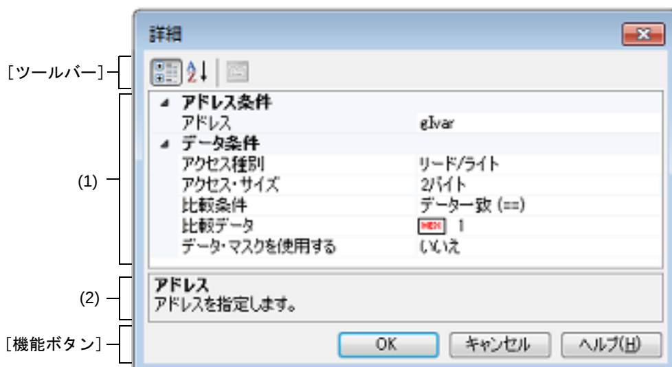
図 A.37 詳細 ダイアログ (アクセス・イベント)【E1】【E20】【EZ Emulator】【COM Port】
