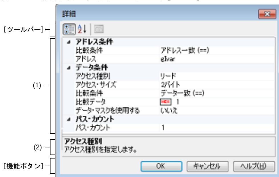
図 A.36 詳細 ダイアログ (アクセス・イベント)【IECUBE】
