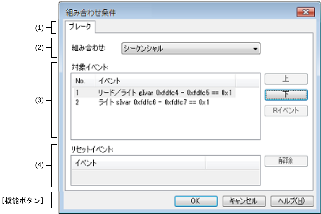
図 A.32 組み合わせ条件 ダイアログ
