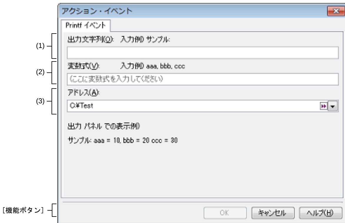
図 A.22 アクション・イベント ダイアログ：[Printf イベント] タブ
