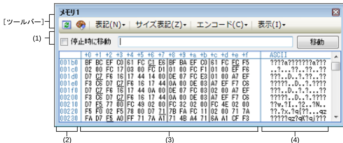
図 A.5 メモリ パネル
