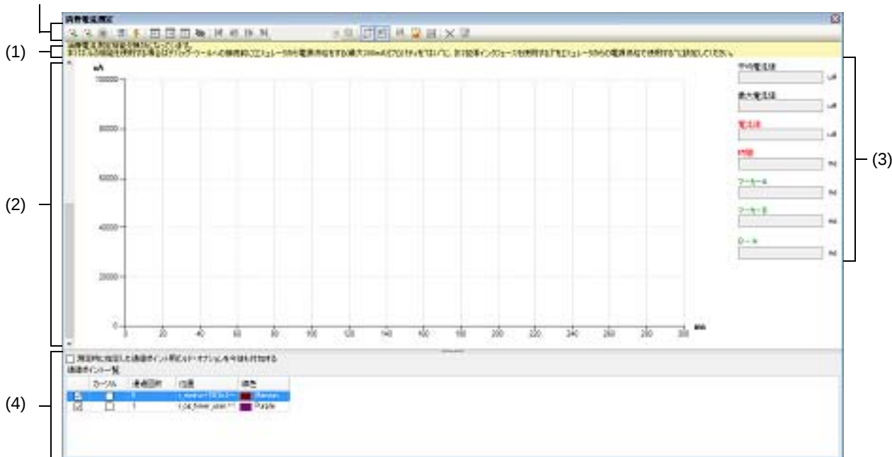
図 A.44 消費電流測定 パネル
