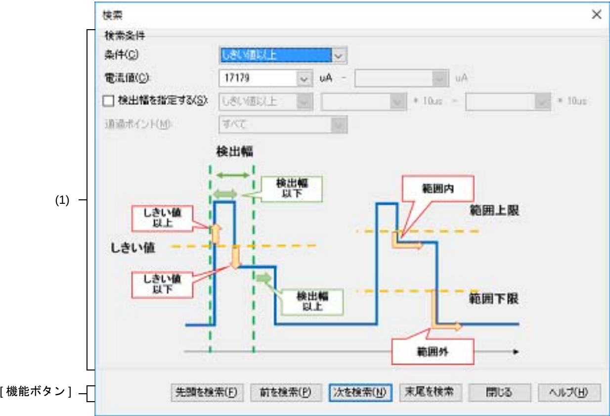
図 A.48 消費電流測定検索 ダイアログ
