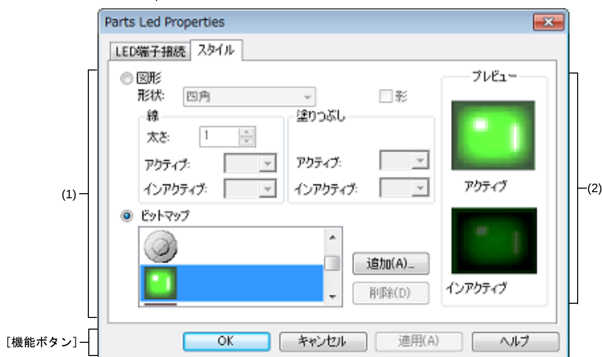
図 A.75 Parts Led Properties ダイアログ : [スタイル] タブ
