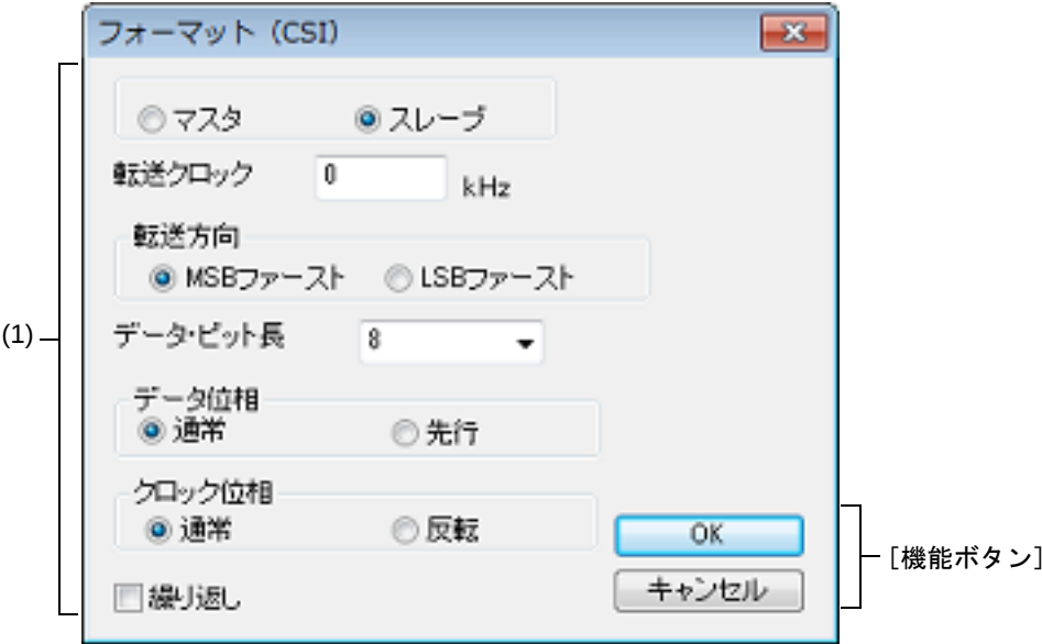
図 A.92 フォーマット（CSI）ダイアログ
