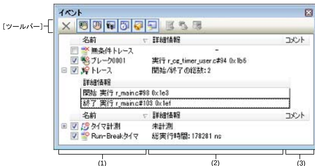
図 A.17 イベント パネル
