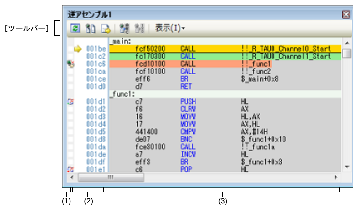
図 A.8 逆アセンブル パネル（コード・カバレッジ測定結果を表示した場合）
