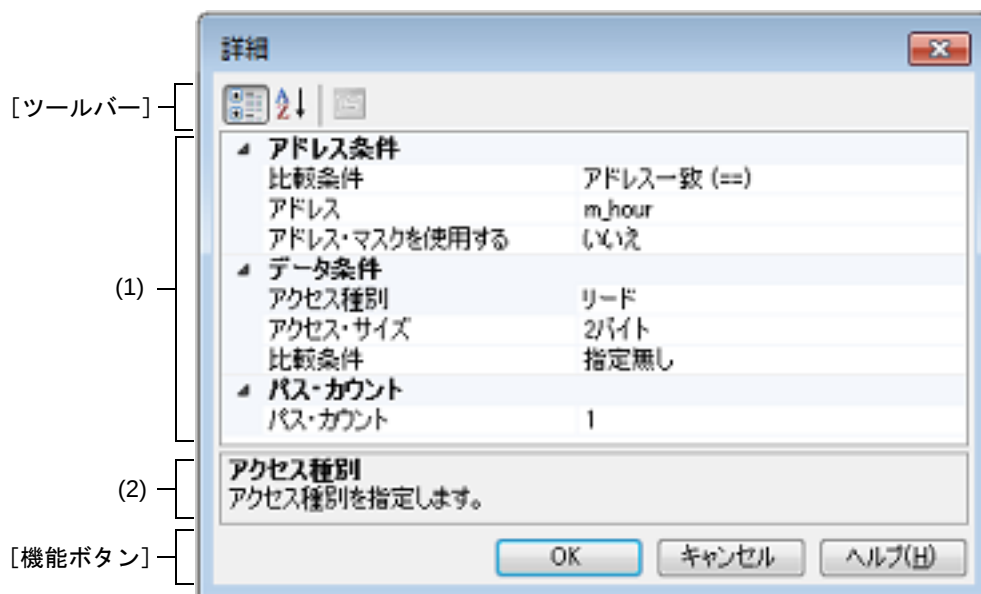
図 A.38 詳細 ダイアログ (アクセス・イベント) 【シミュレータ】
