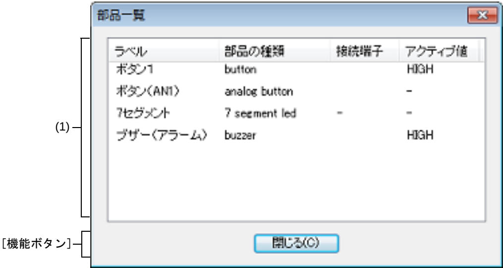
図 A.89 部品一覧 ダイアログ
