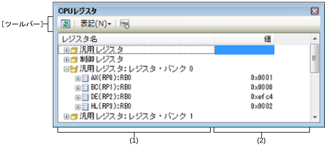
図 A.10 CPU レジスタ パネル
