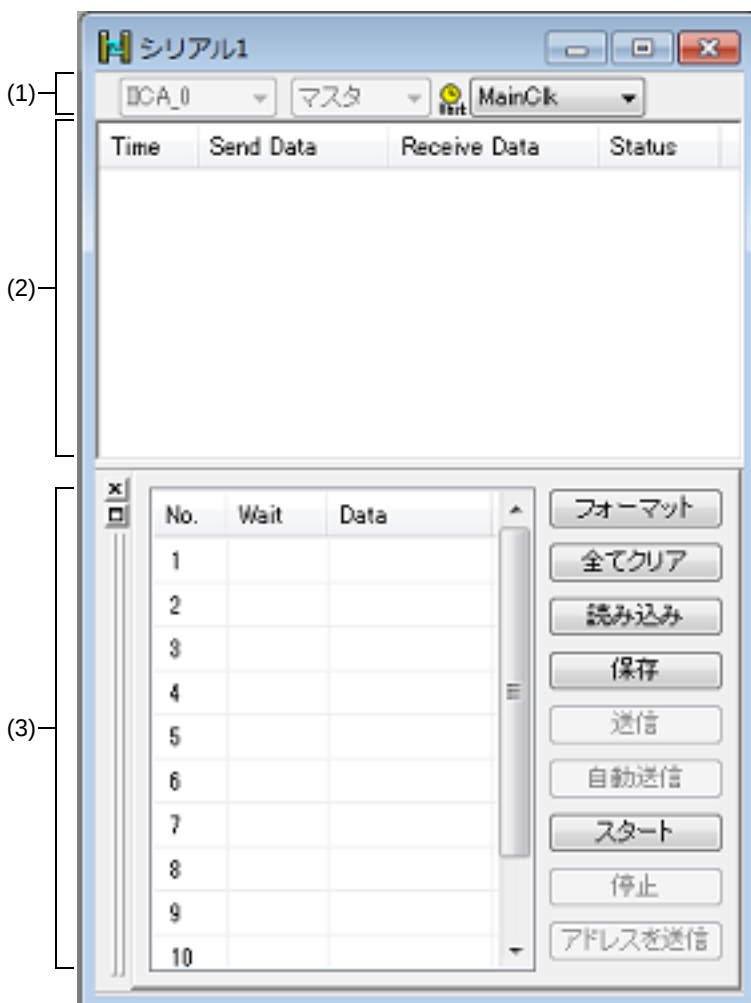
図 A.90 シリアル ウィンドウ
