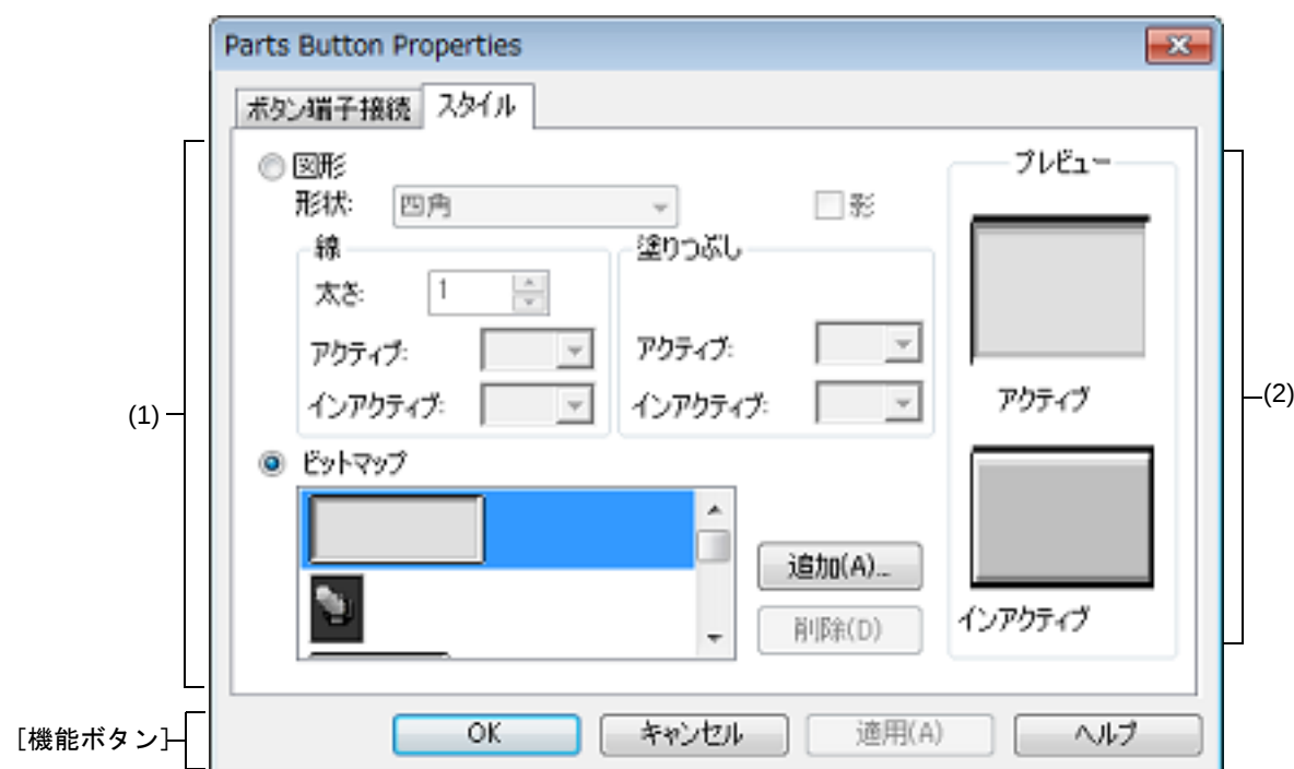
図 A.63 Parts Button Properties ダイアログ : [スタイル] タブ
