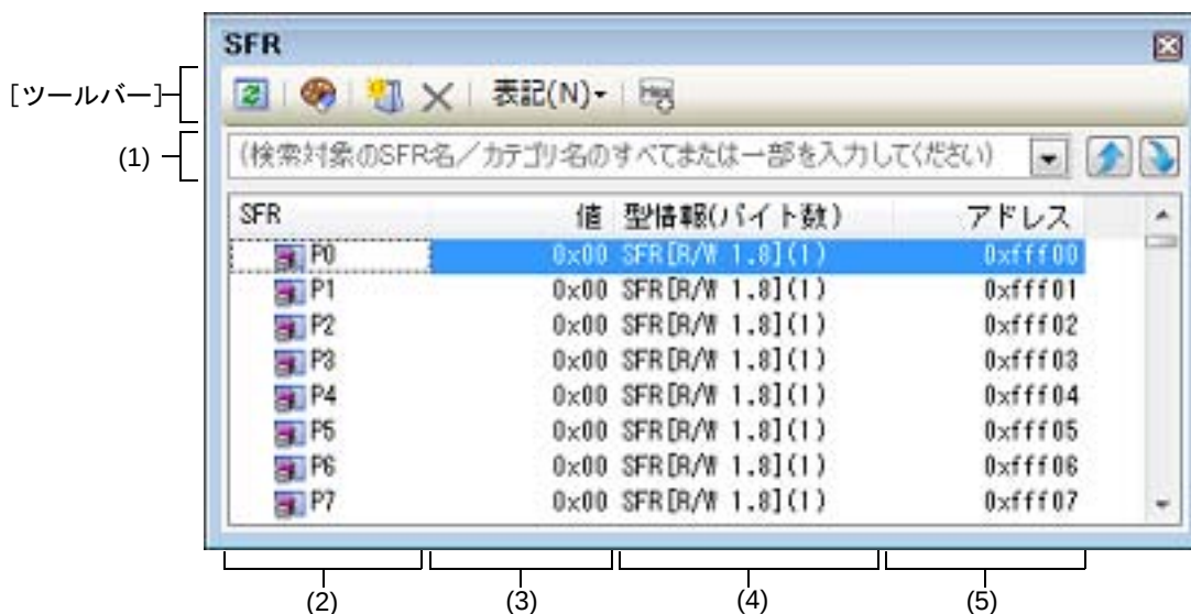
図 A.11 SFR パネル
