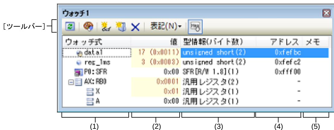
図 A.13 ウォッチ パネル
