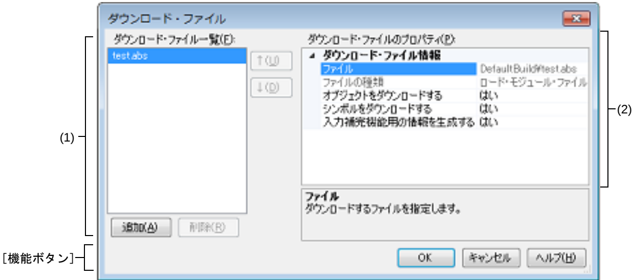
図 A.20 ダウンロード・ファイル ダイアログ
