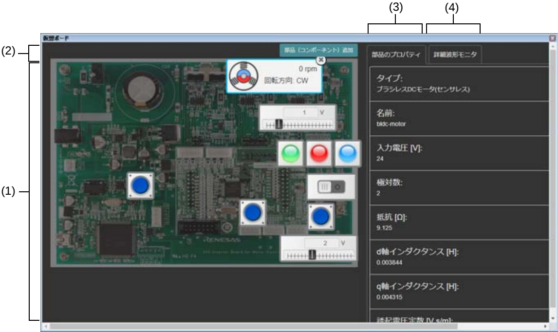
図 A.50 仮想ボード パネル【シミュレータ】
