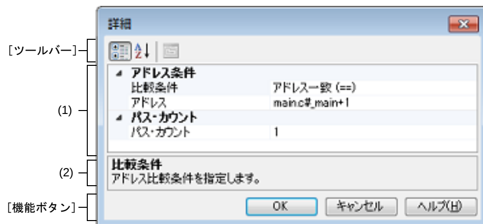
図 A.34 詳細 ダイアログ（実行イベント）【E1】【E20】【EZ Emulator】【COM Port】
