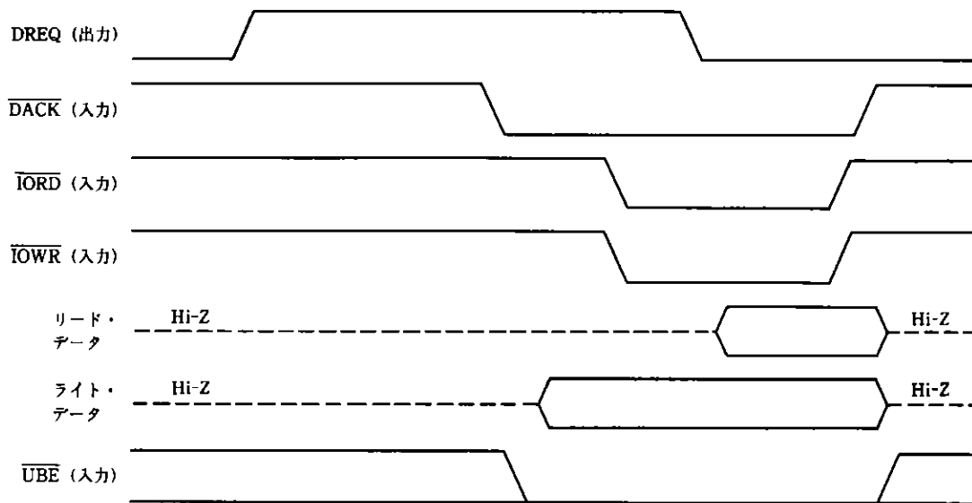
図7-12a 外部DMAコントローラとの読み出し/書き込みタイミング (ワード・モード)
