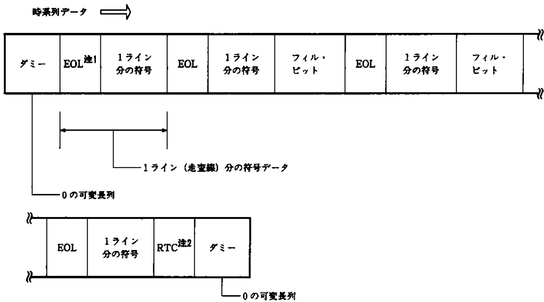
図6-3 MH方式における符号データ・フォーマット
