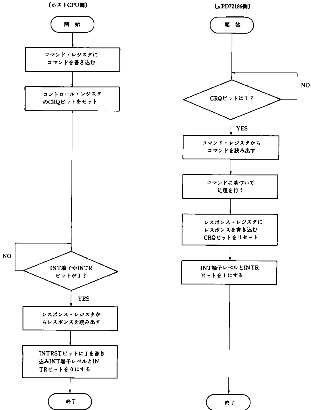
図 7-4 μPD72186の制御フロー
