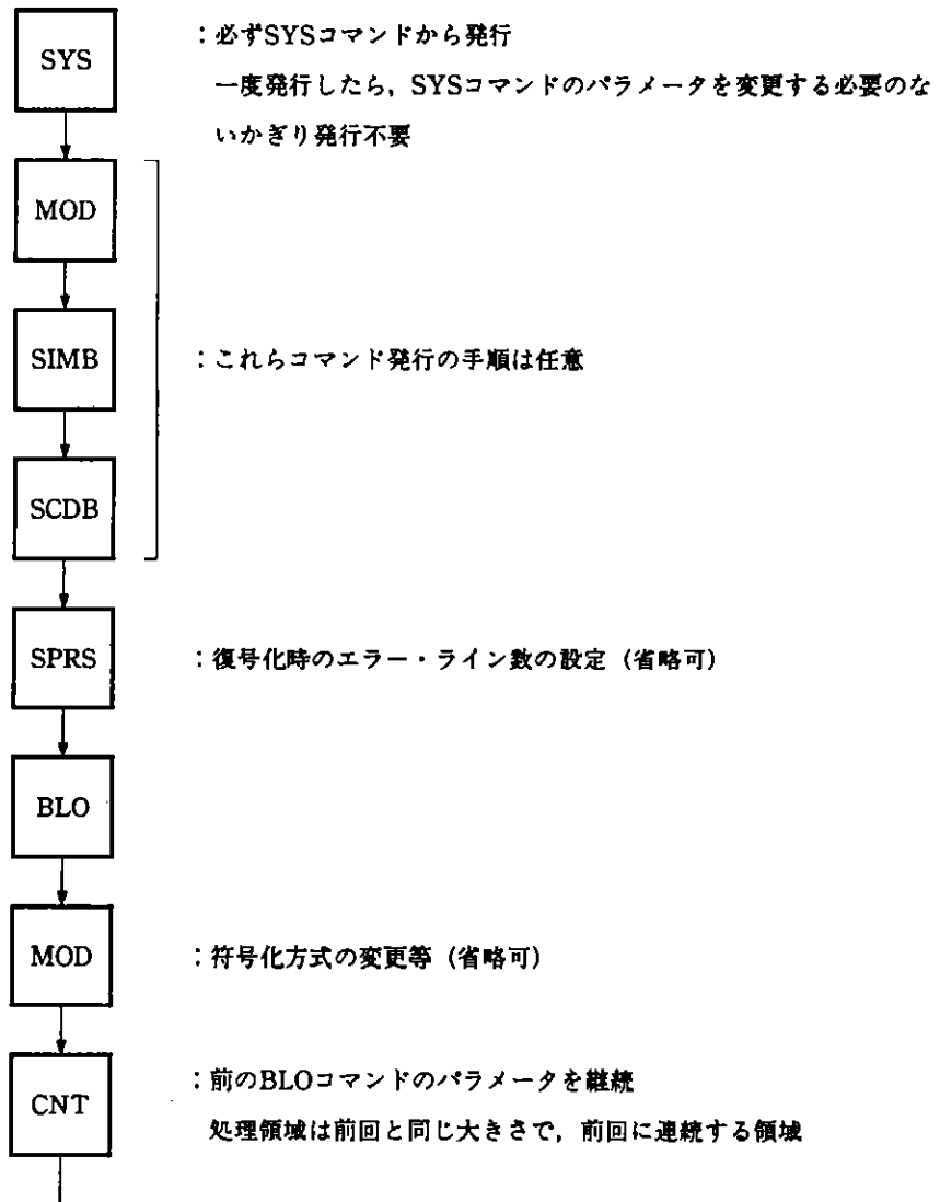
図8-1 ブロック・モードの基本フロー
