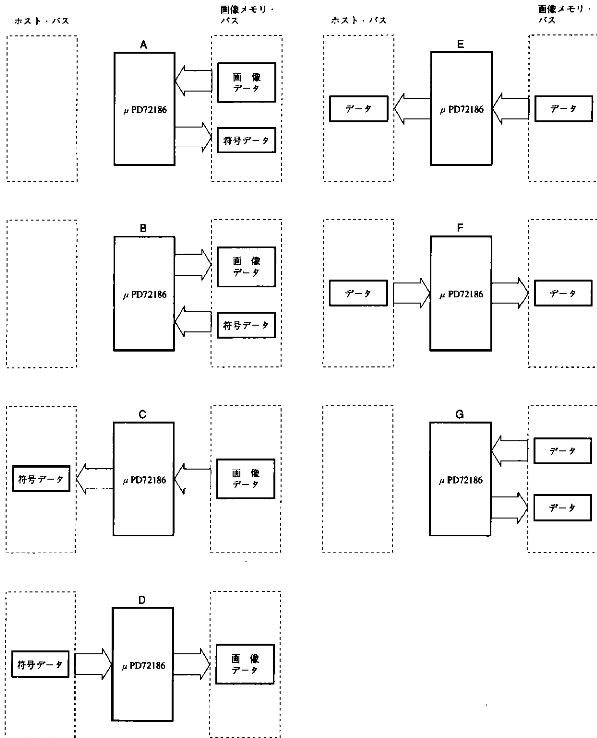
図 5-1 \mu PD72186の処理形態
