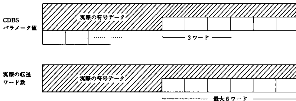
図7-2 CDBSパラメータ値の設定が「符号データ数 + 3ワード」より大きい場合
