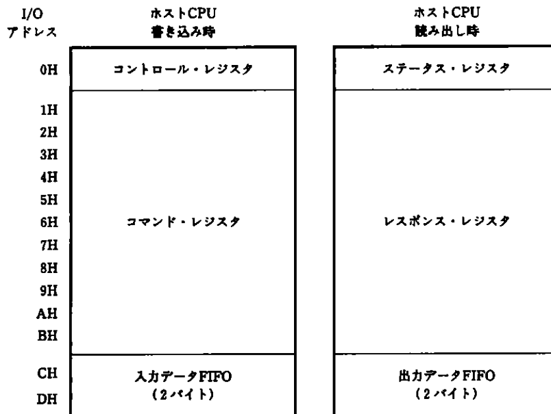
図7-5 レジスタ構成
