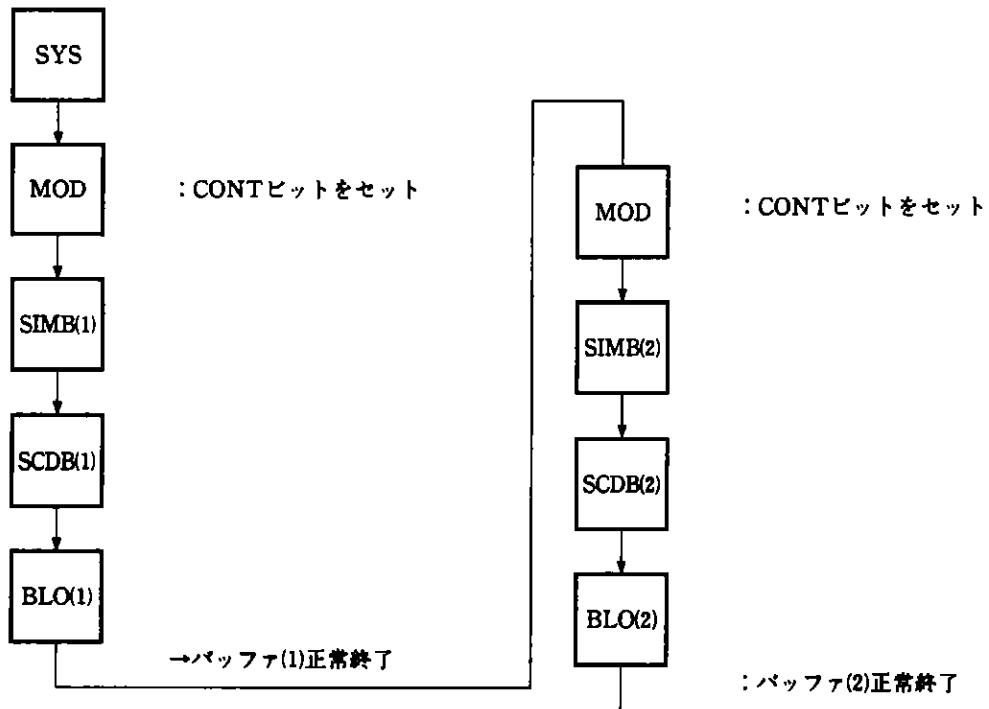
図8-5 時分割による複数処理
