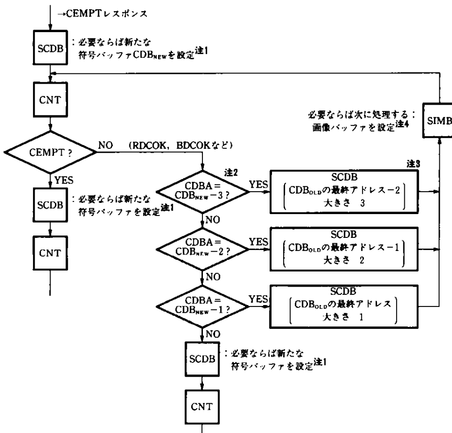
図8-4 符号バッファ・エンプティ（掃き出しモード時）後の符号バッファ再設定
