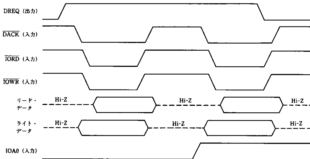
図7-12b 外部DMAコントローラとの読み出し/書き込みタイミング (バイト・モード)
