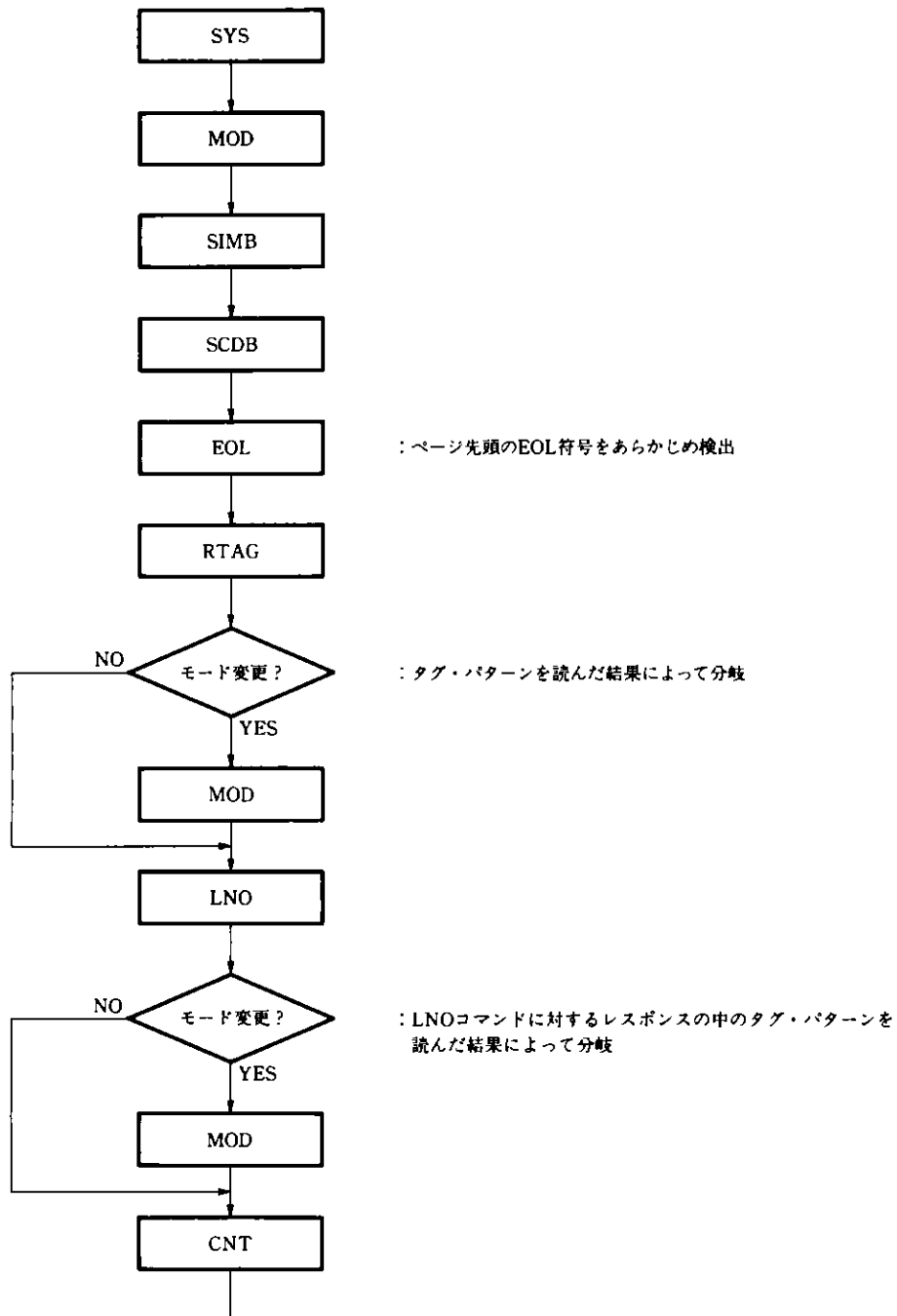
図8-8 ライン・モードの基本フロー（復号化処理）
