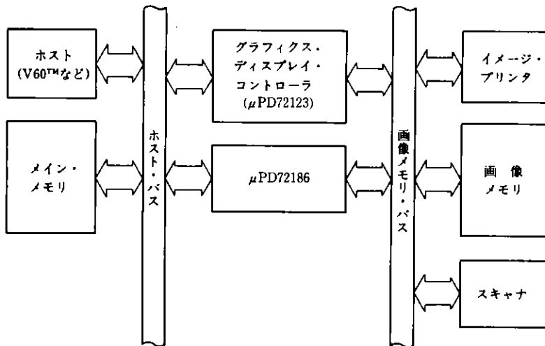
図2-2 ハイ・エンド・タイプの構成例
