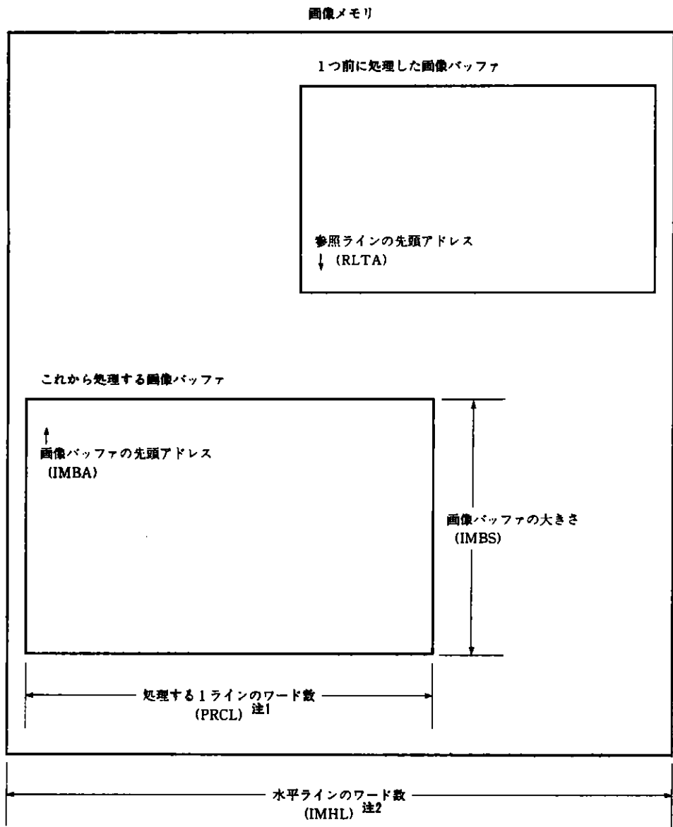
図 8-21 画像メモリとパラメータ (符号化/復号化)
