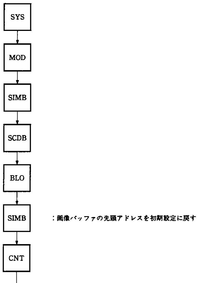
図8-2 画像バッファのサイクリックな使用
