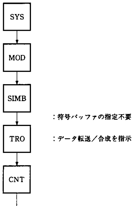
図8-11 データ転送の基本フロー
