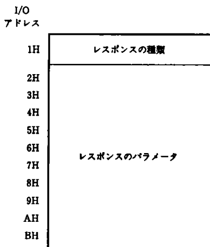
図7-9 レスポンス・レジスタ
