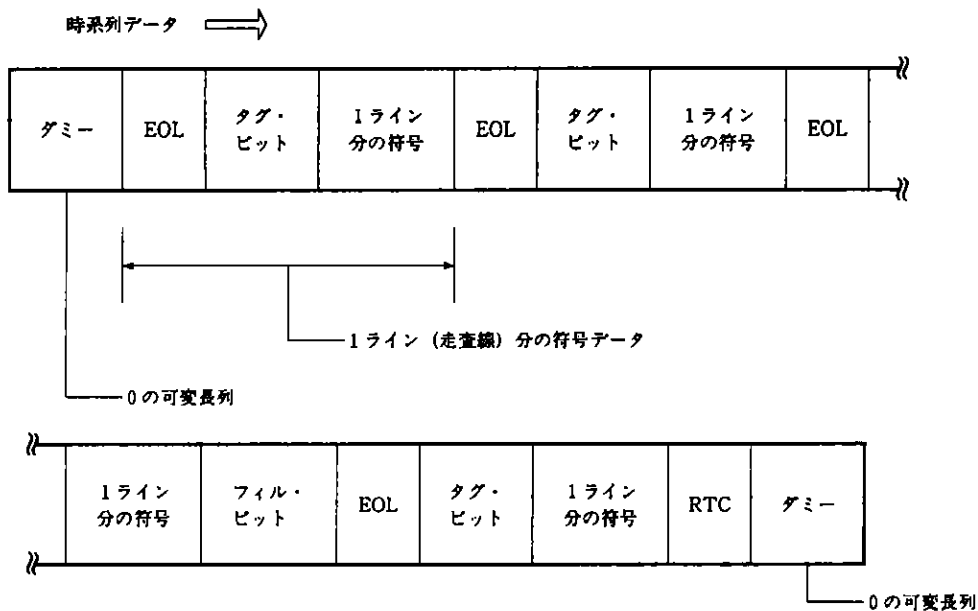
図6-4 MR方式における符号データ・フォーマット
