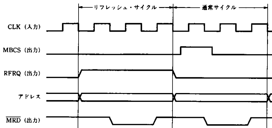
図7-14 リフレッシュ・タイミング
