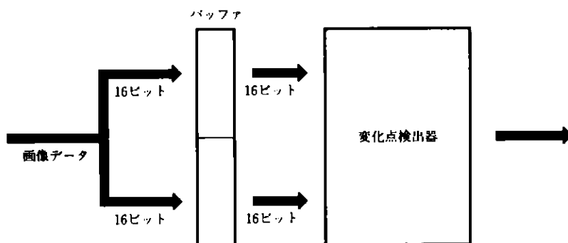
図7-16 μPD72186の内部ブロック図
