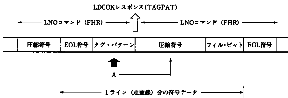
図8-9 1ラインの符号データ・フォーマット
