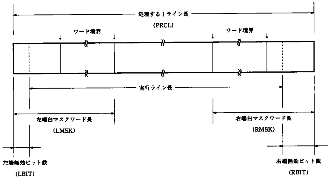
図 8-34 実際に処理するラインとパラメータ
