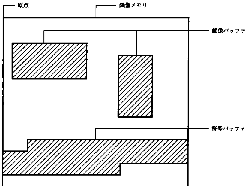
図6-1 画像メモリと画像／符号バッファ
