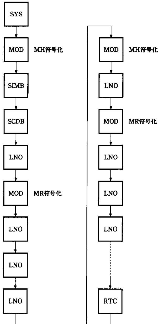
図8-7 ライン・モードでのMR符号化の基本フロー（K=4の場合）
