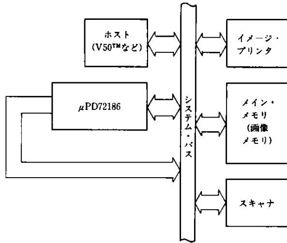
図2-1 ロウ・エンド・タイプの構成例
