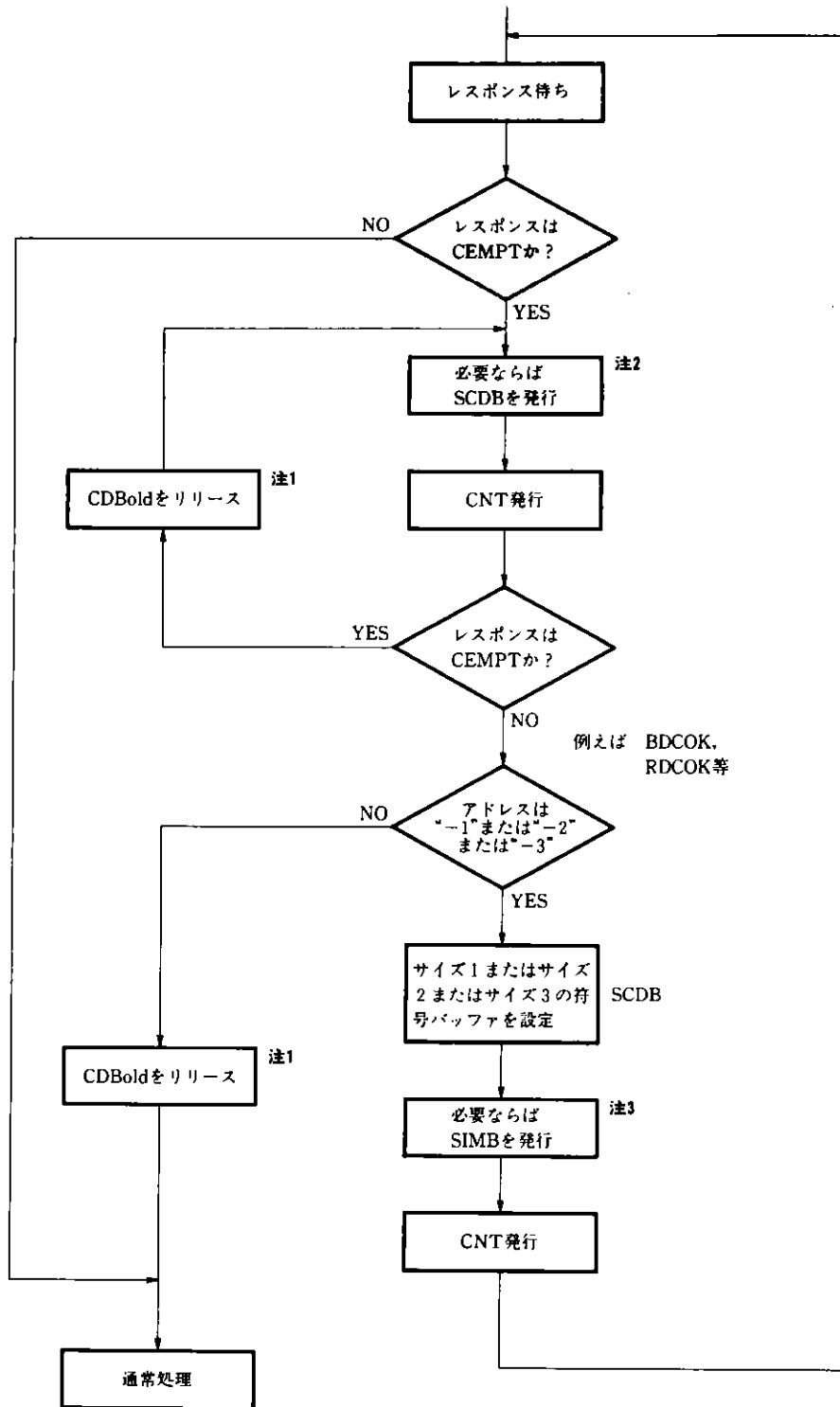
図 8-81 掃き出しモードでのCEMPT処理(2)
