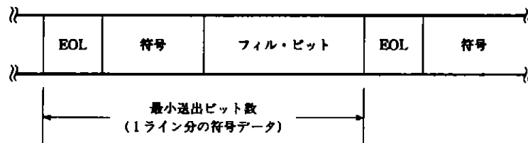
図6-6 最小送出ビット数
