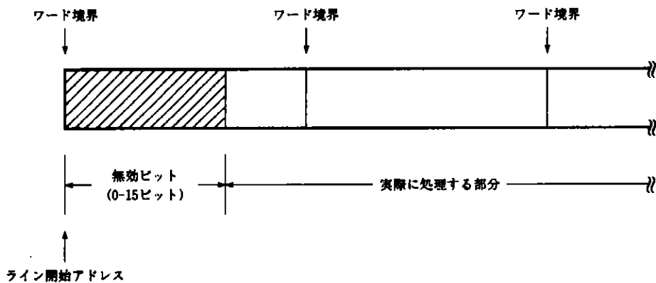
図5-5 ビット・バウンダリ処理 (ワード単位)
