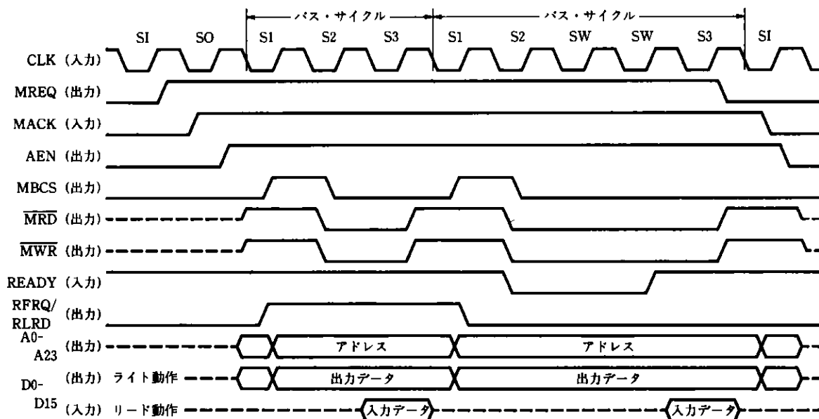
図7-13 DMA転送タイミング
