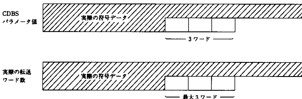
図7-3 CDBSパラメータ値の設定が「符号データ数 + 3ワード」の場合
