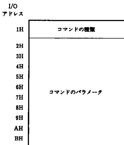
図7-8 コマンド・レジスタ
