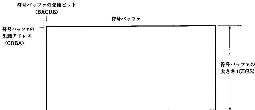
図 8-28 符号バッファ内のビットの位置
