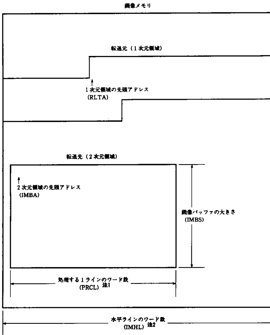
図 8-23 画像メモリとパラメータ (データ転送: 1次元領域→2次元領域)
