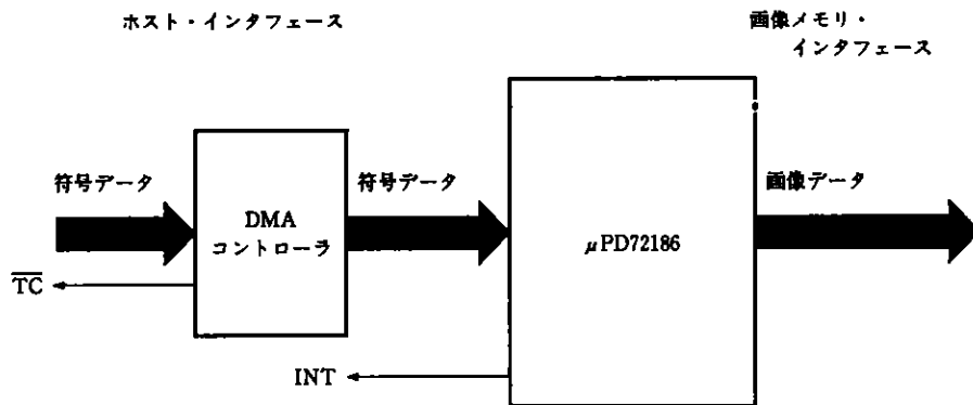
図7-1 外部DMAを用いたシステム例
