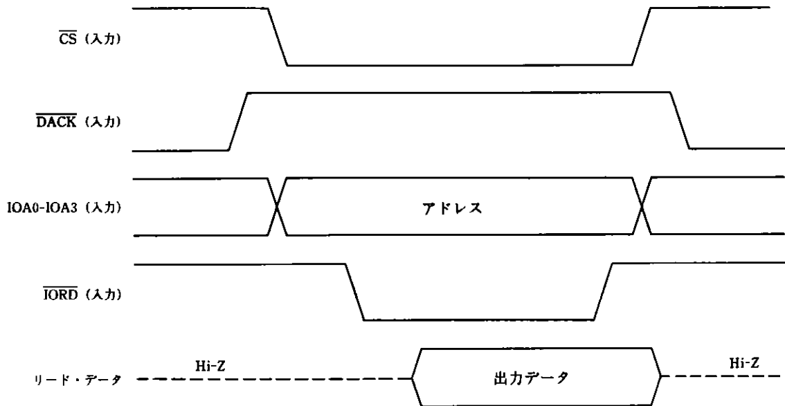
図7-11a \mu PD72186からの読み出しタイミング
