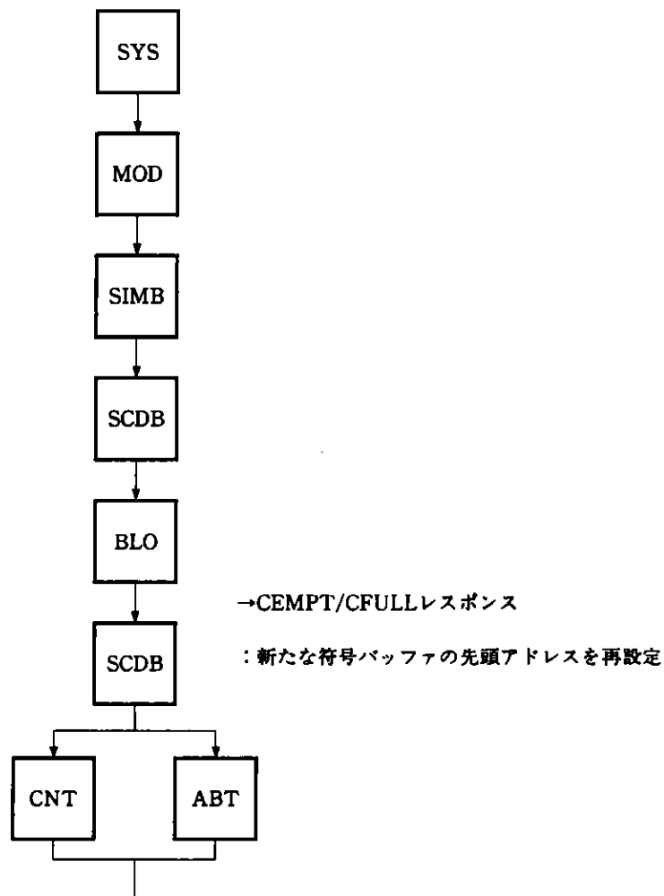
図8-3 符号バッファ・フル/エンプティ（継続処理モード時）後の符号バッファ再設定
