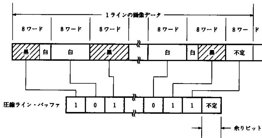
図 8-73 圧縮ライン・バッファ
