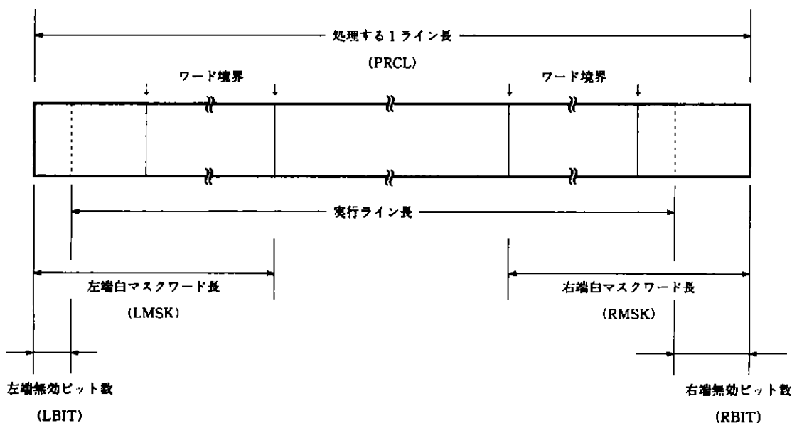
図 8-34 実際に処理するラインとパラメータ
