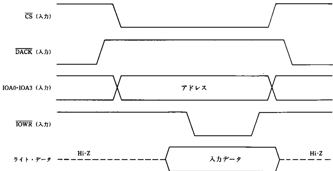
図7-11b \mu PD72186への書き込みタイミング
