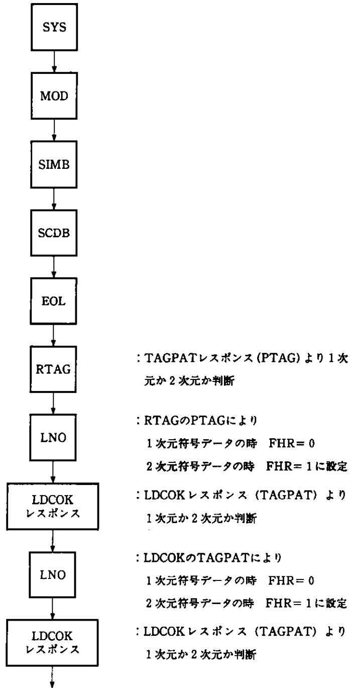
図 8-10 ライン・モードでの基本フロー (MR復号化処理)
