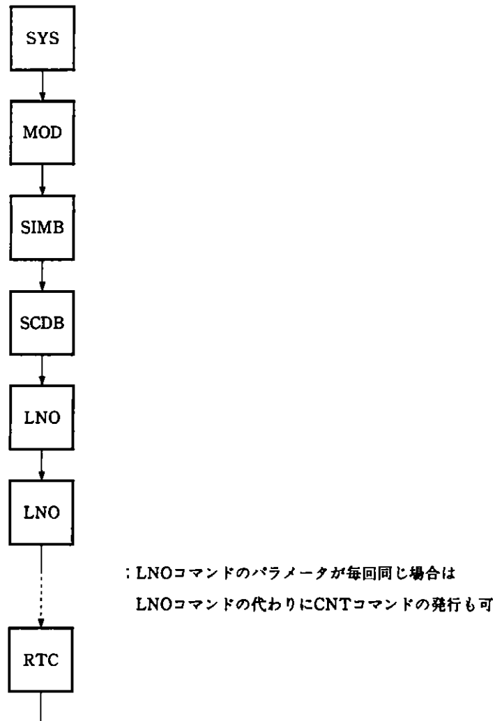
図8-6 ライン・モードの基本フロー（符号化処理）
