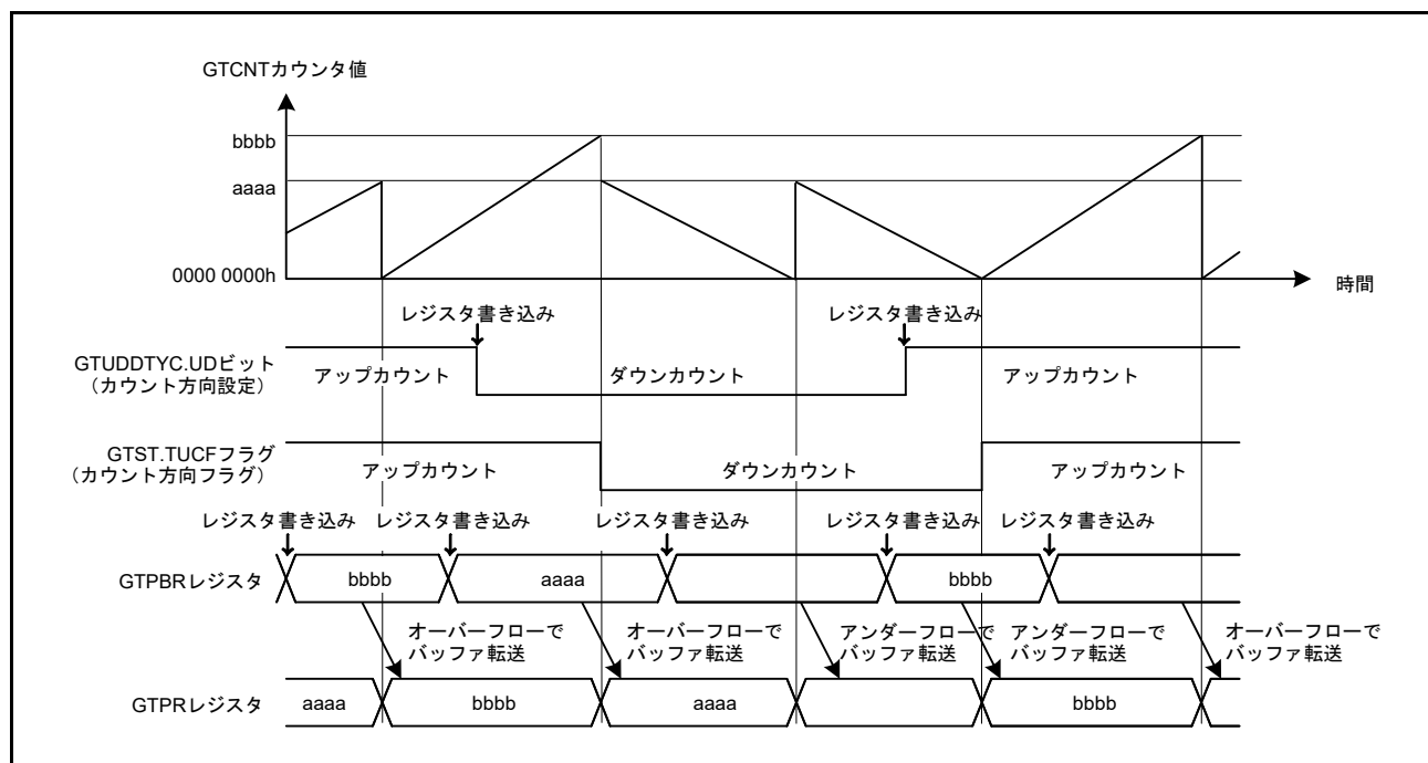
図 21.45 カウント方向切り替え機能の動作例（バッファ動作時）
