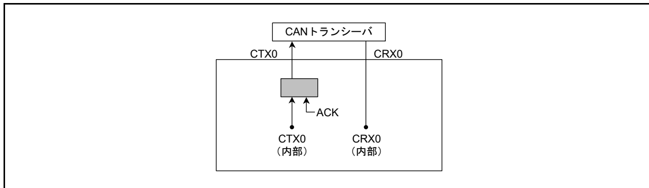
図 29.7 セルフテストモード 0 選択時の接続
