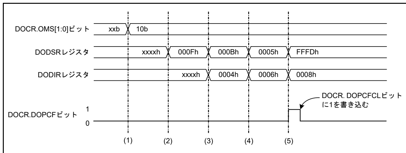
図 41.4 データ減算モードの動作例
