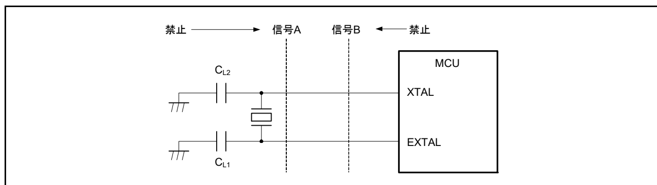
図 9.8 発振回路部のボード設計に関する信号のルーティング (メインクロック発振器の場合、サブクロック発振器も同様)
