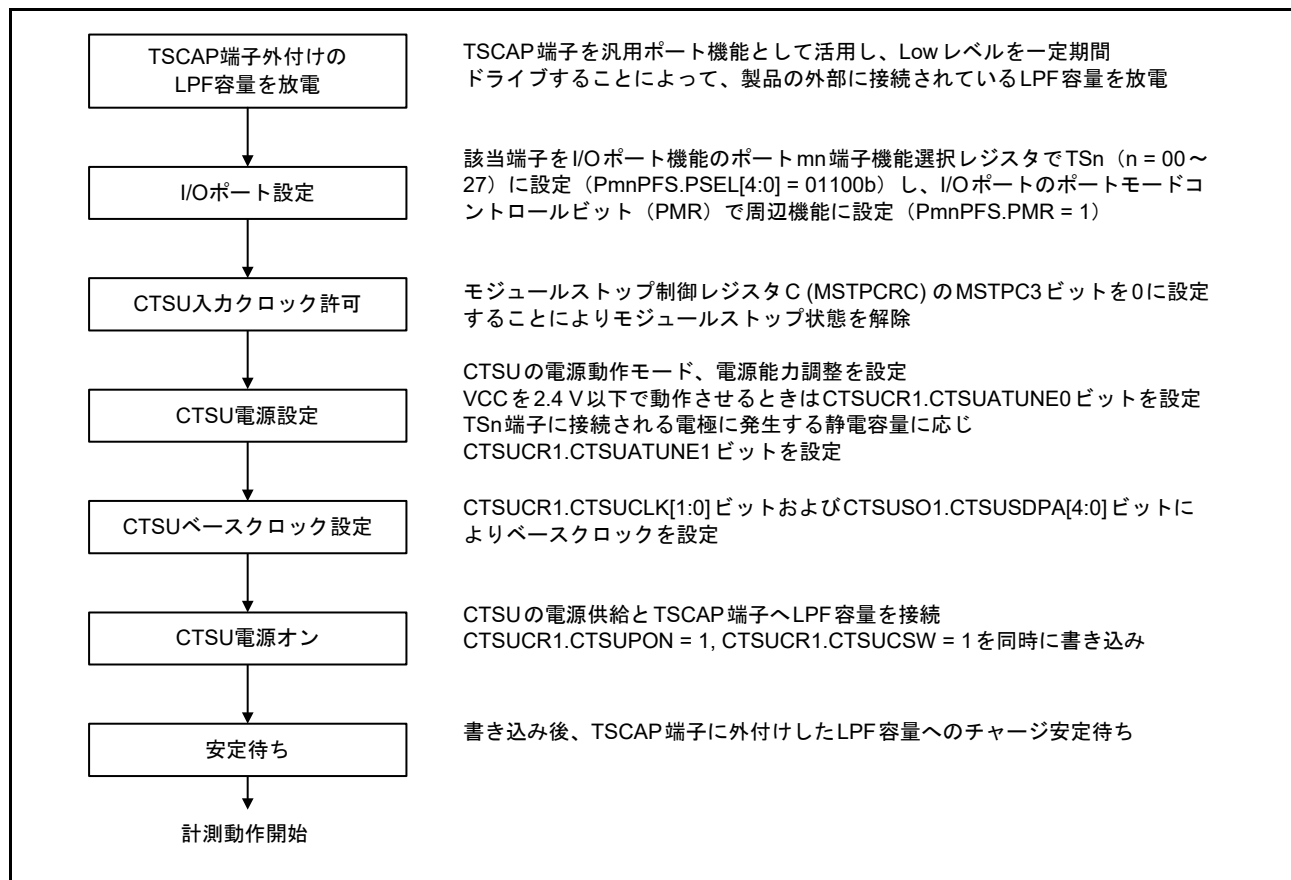
図 40.9 CTSU 初期設定フロー
