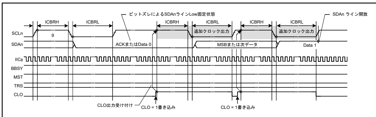
図 28.49 SCL クロック追加出力機能 (CLO ビットの使用)
