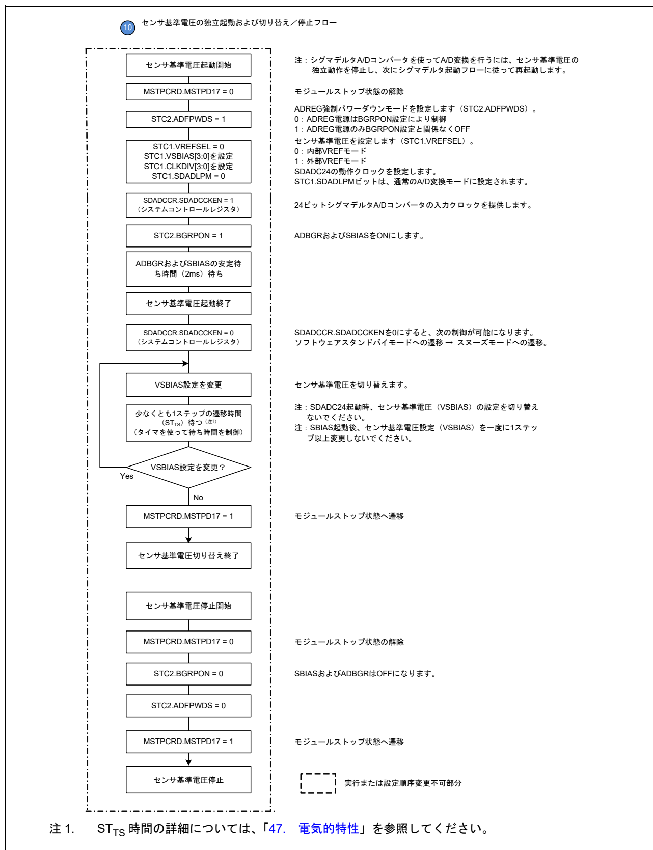
図 33.32 センサ基準電圧の独立起動および切り替え/停止フロー
