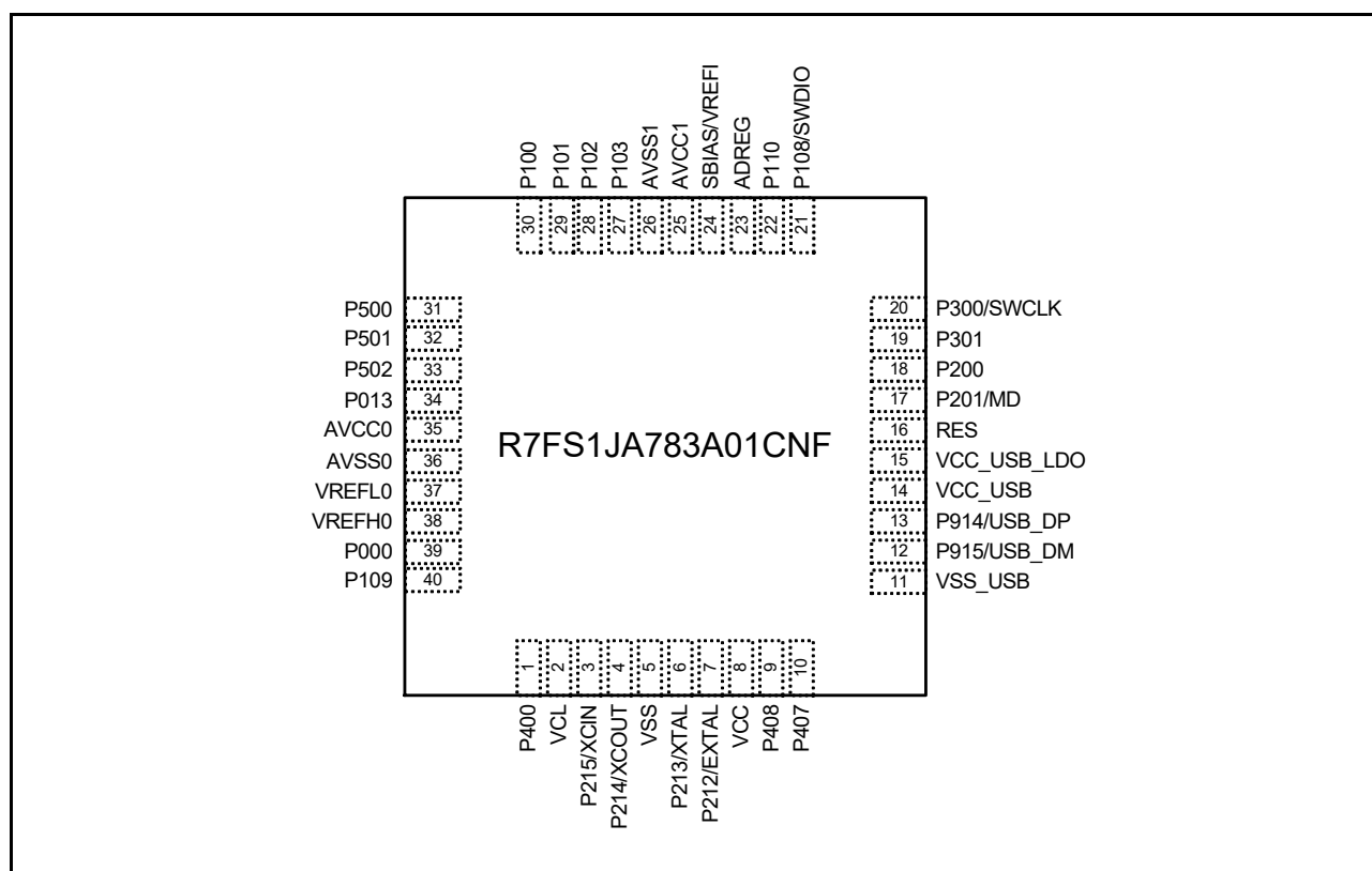
図 1.5 40-pin LQFP のピン配置
