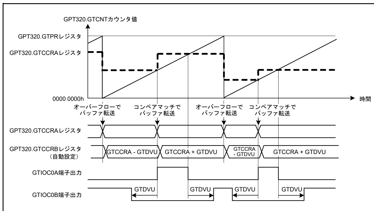
図 21.39 デッドタイム自動設定機能の動作例 (のこぎり波ワンショットパルスモード、アップカウント、アクティブ High の場合)
