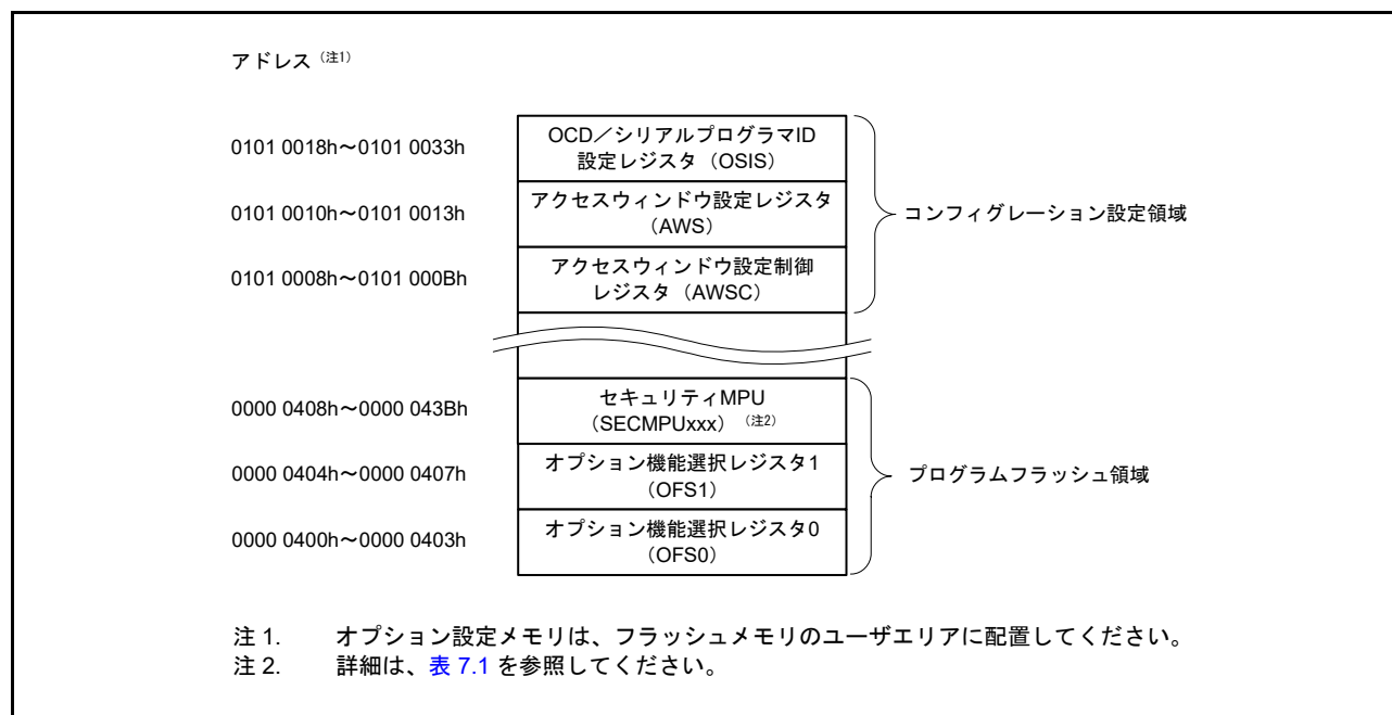
図 7.1 オプション設定メモリの領域
