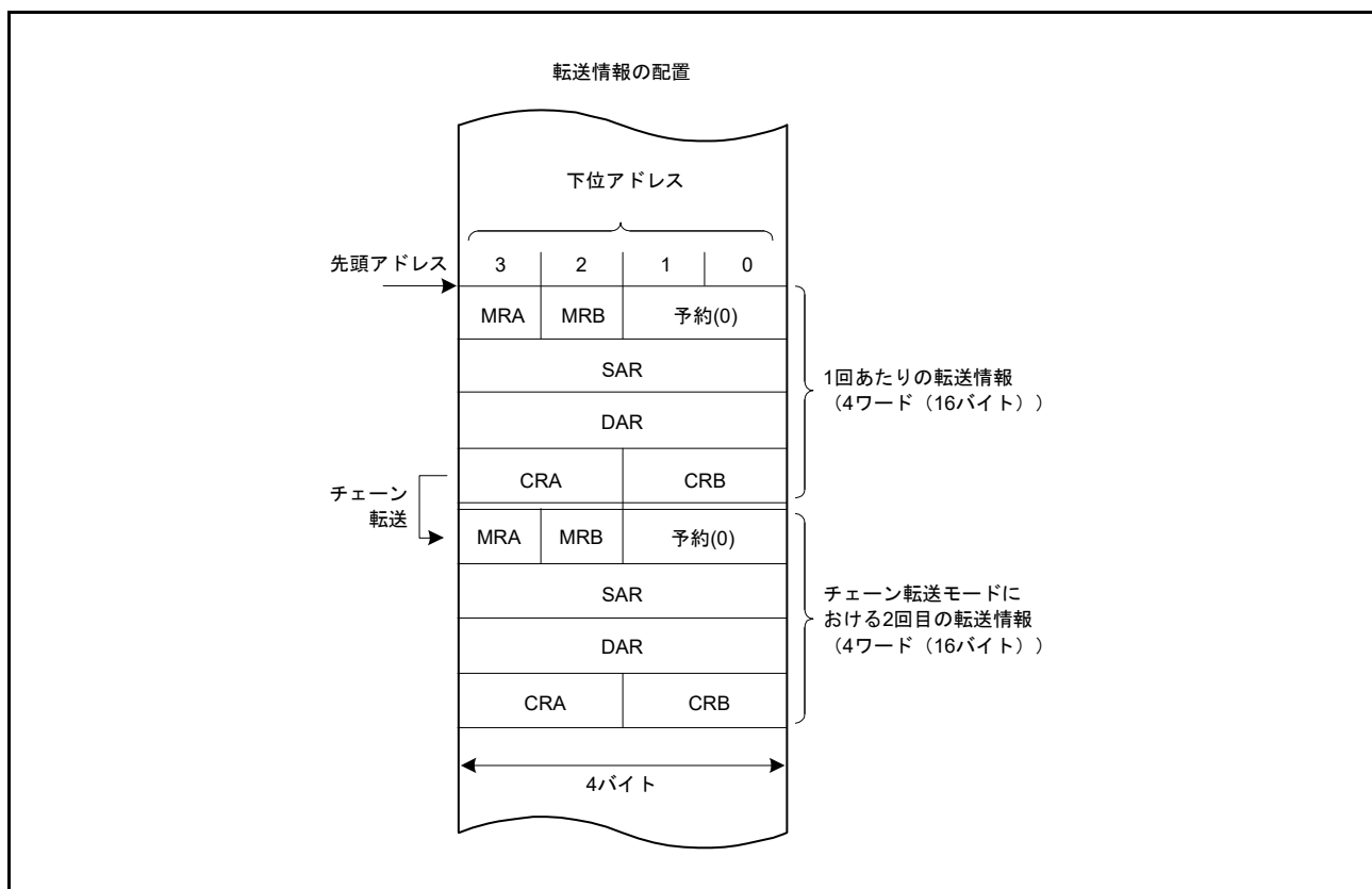
図 16.3 SRAM 領域上の転送情報の配置
