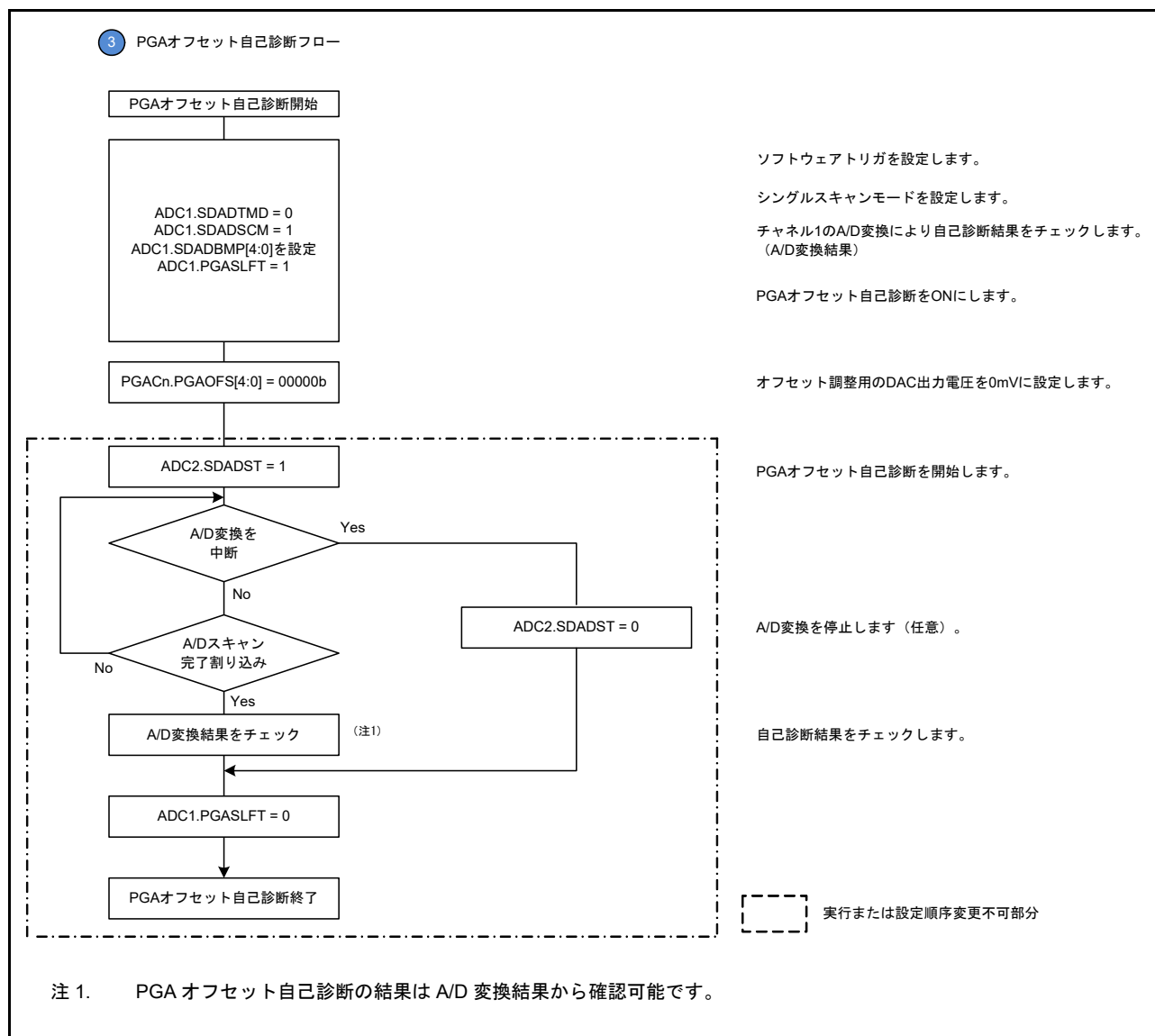
図 33.25 PGA オフセットの自己診断フロー
