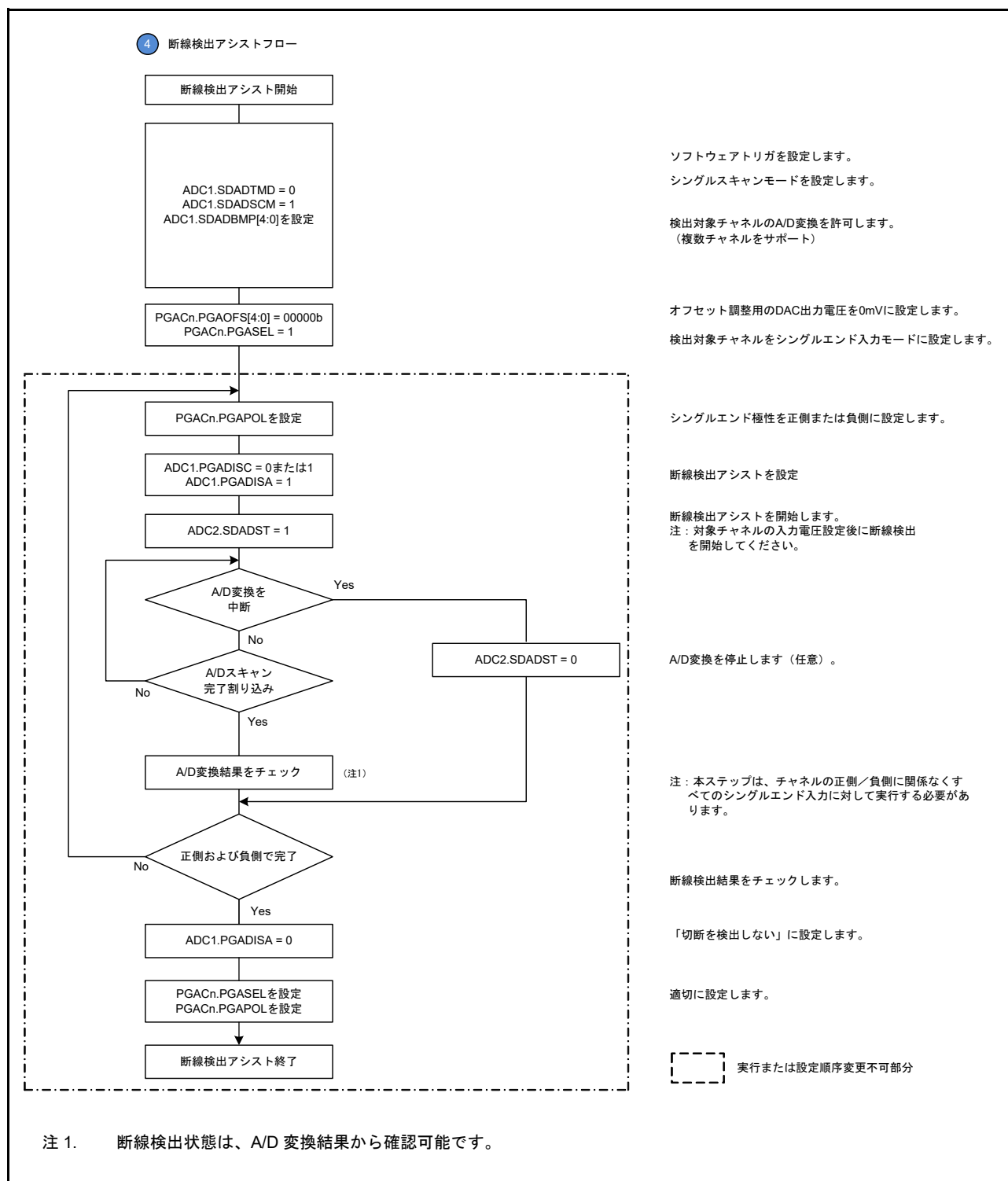
図 33.26 断線検出アシストフロー
