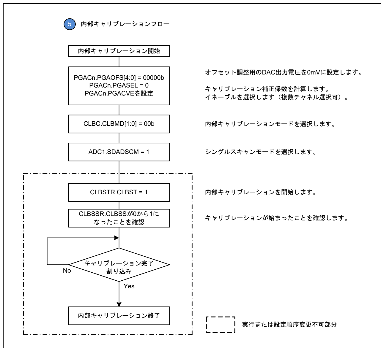
図 33.27 内部キャリブレーションフロー
