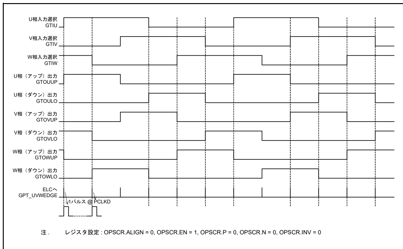
図 21.78 6 相レベル出力動作例
