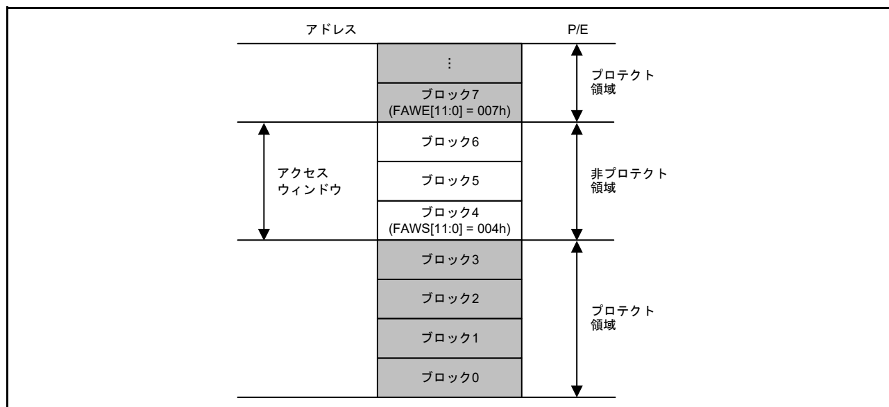
図 7.2 アクセスウィンドウの概要
