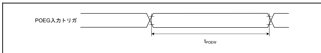
図 47.37 POEG 入力トリガタイミング
