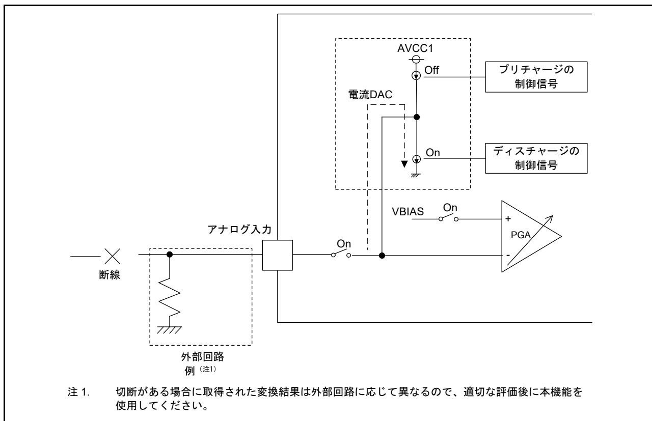
図 33.20 シングルエンド入力モード（負側）でディスチャージ選択時の切断検出例
