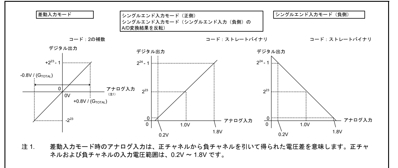
図 33.11 SDADC24 用入力電圧および A/D 変換結果
