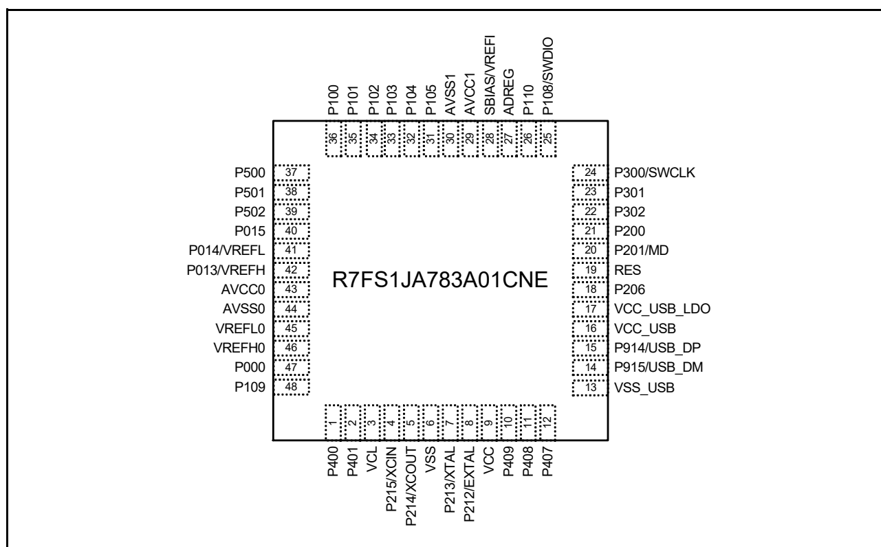
図 1.4 48-pin QFN のピン配置
