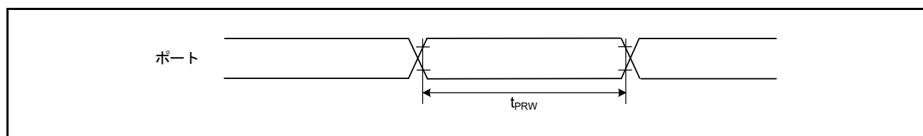
図 47.36 I/O ポート入力タイミング
