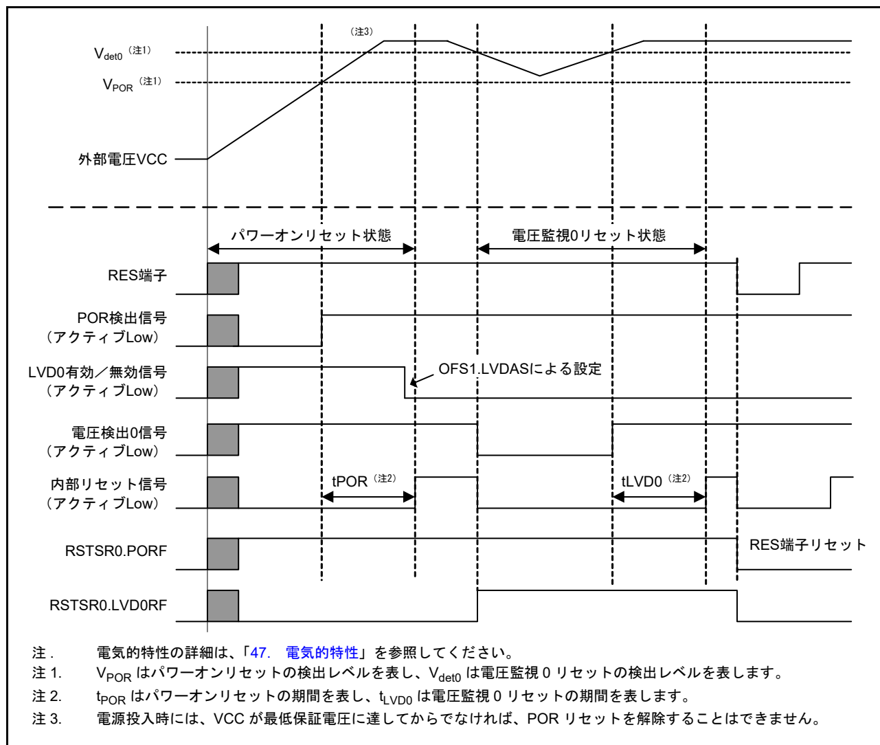
図 8.4 電圧監視 0 リセットの動作例
