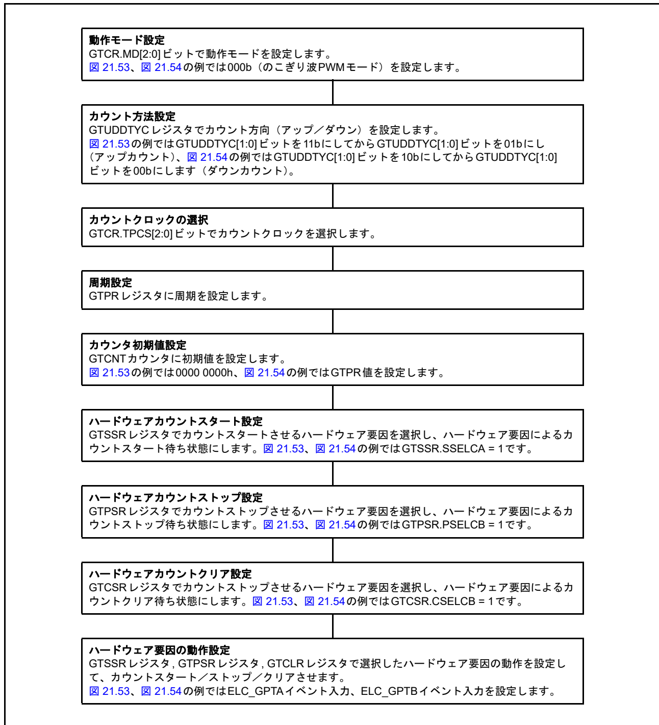
図 21.55 ハードウェア要因によるカウントクリア動作設定例
