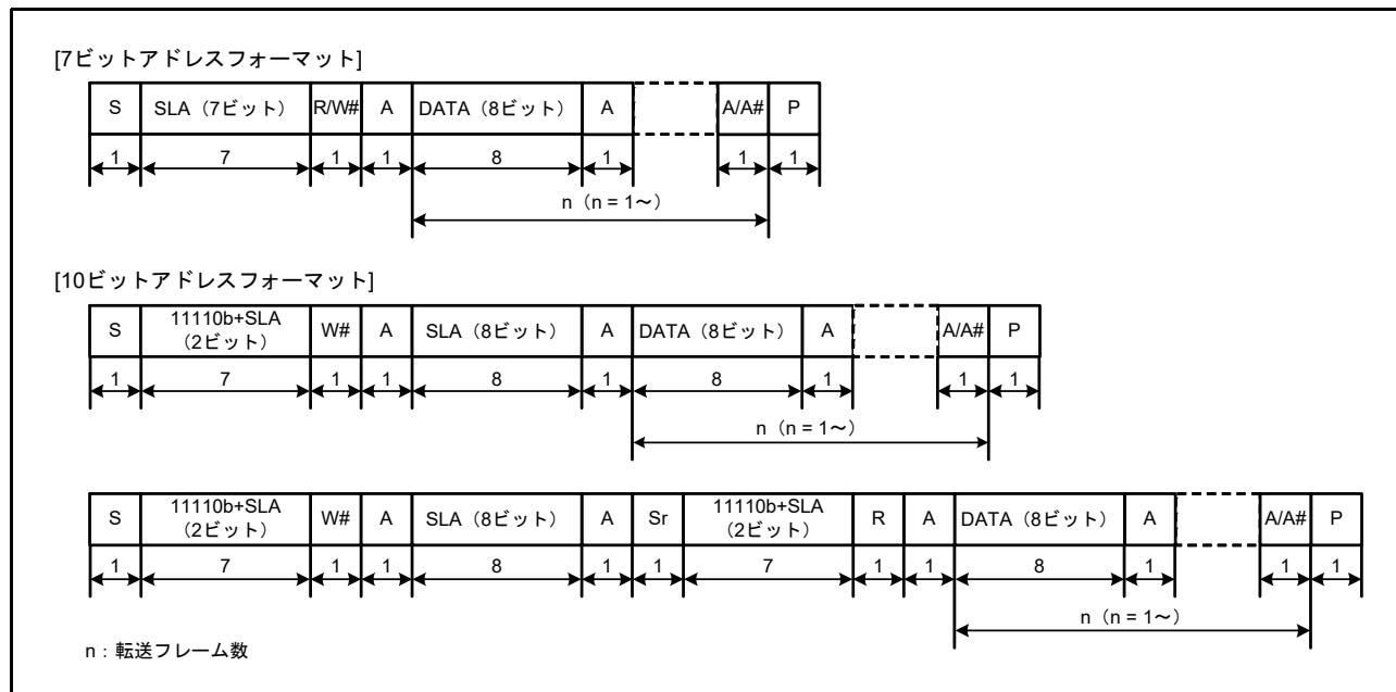
図 28.3 I 2 C バスフォーマット
