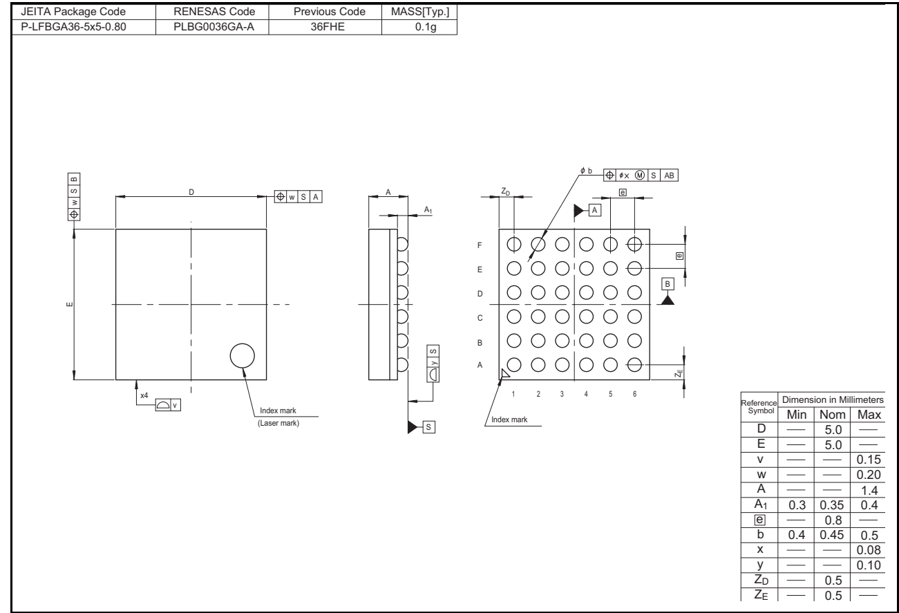
図 2.3 BGA 36 ピン
