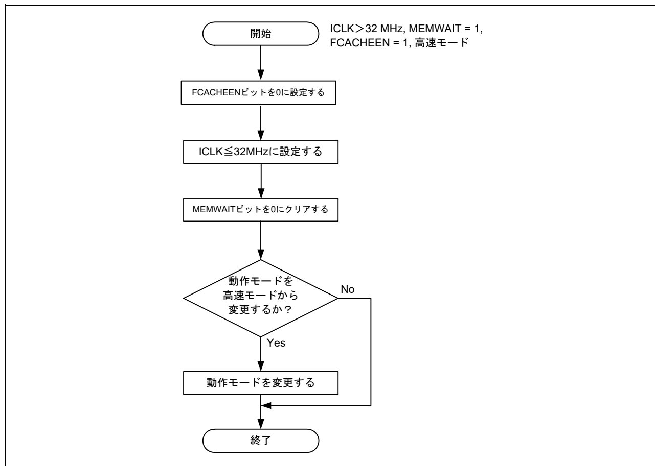
図 9.3 ICLK > 32\text{MHz} の状態から ICLK \leq 32\text{MHz} に設定する場合
