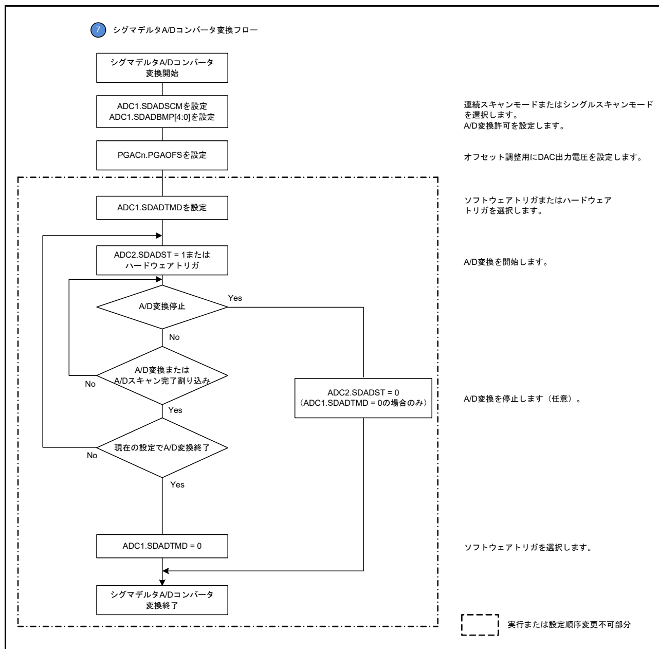
図 33.29 SDADC24 変換フロー
