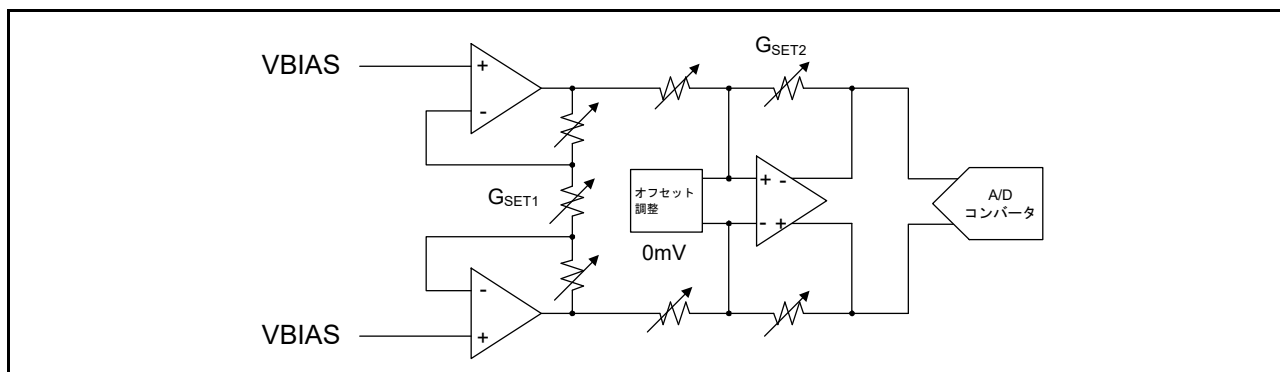
図 33.21 PGA オフセットの自己診断機能構成
