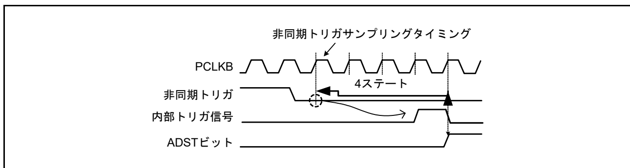
図 32.33 非同期トリガ入力タイミング
