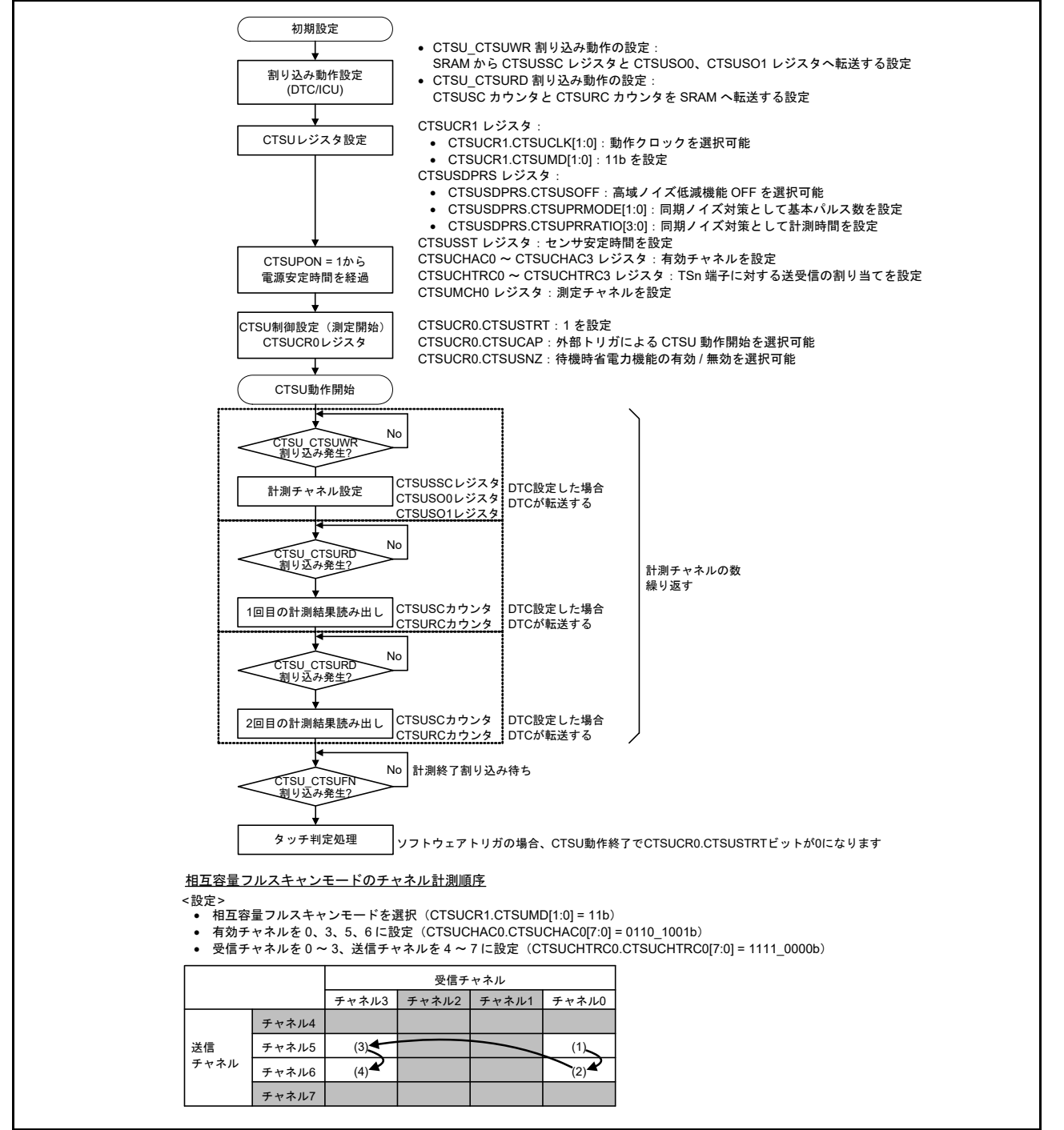
図 40.16 相互容量フルスキャンモードのソフトウェアフローと動作例
