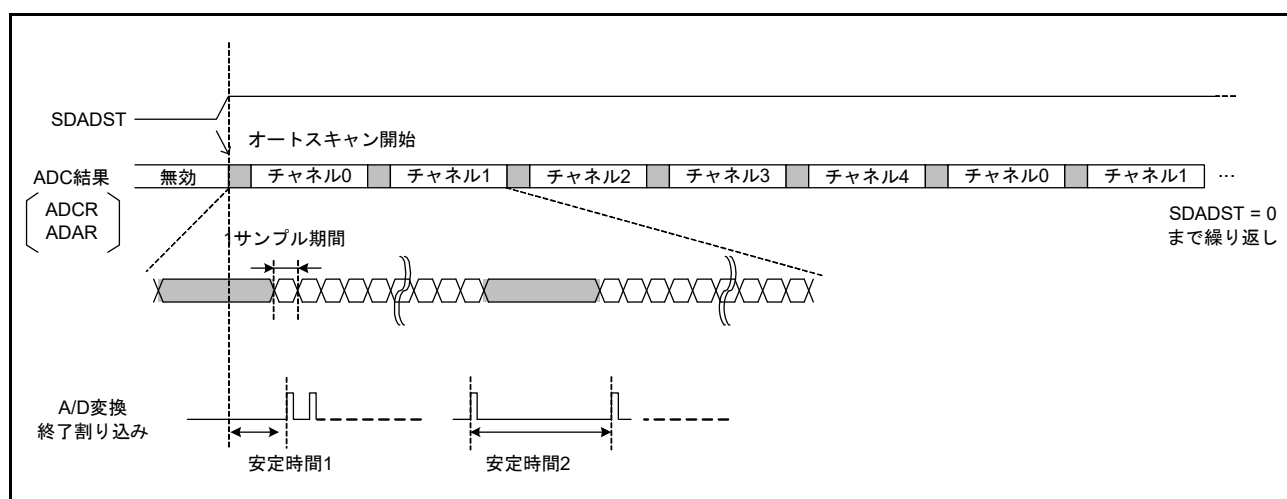
図 33.12 オートスキャンシーケンス
