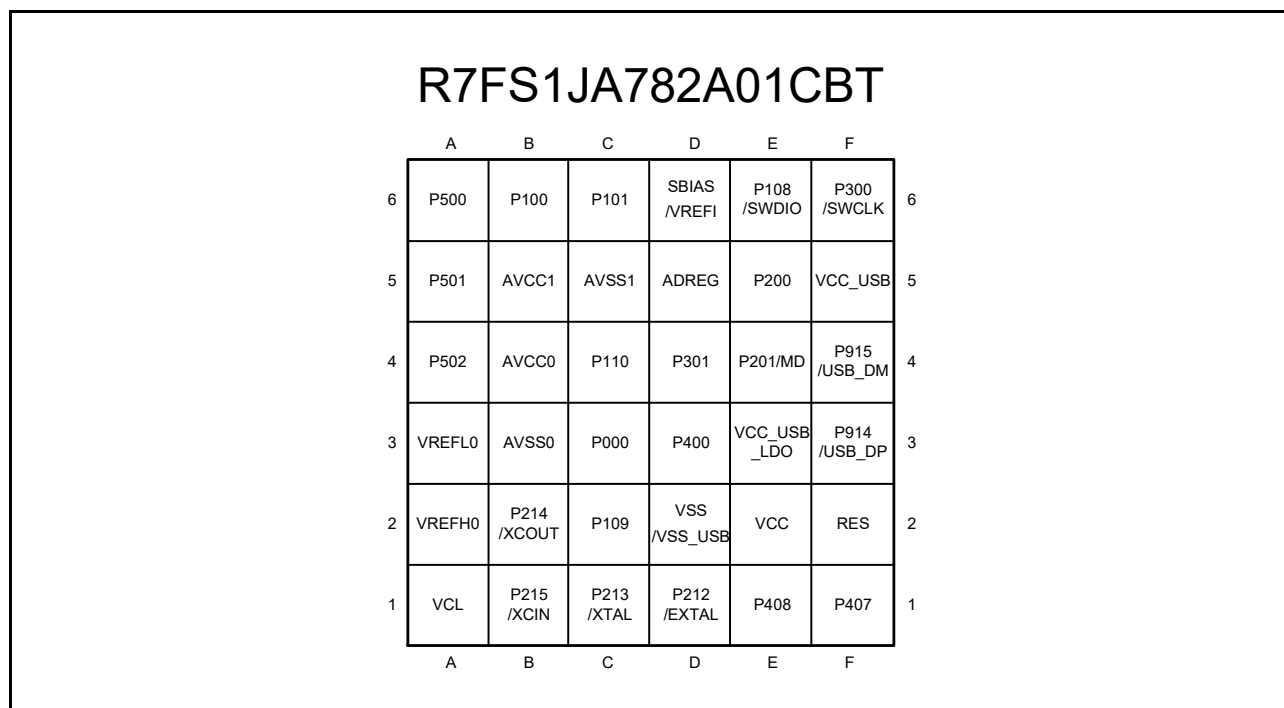
図 1.6 36-pin BGA のピン配置（上面図、パッド側が下面）
