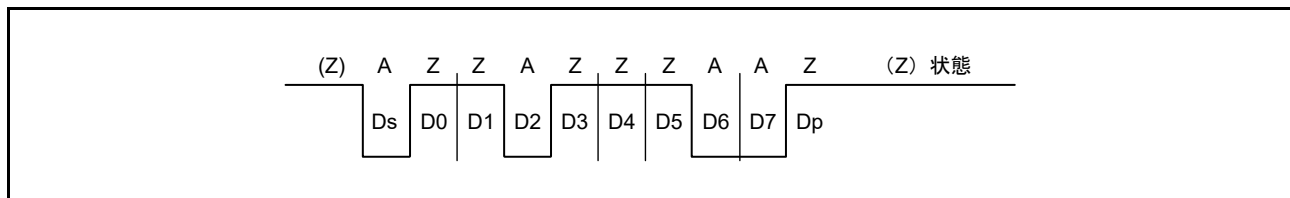
図 27.47 ダイレクトコンベンション (SCMR.SDIR ビット = 0、SCMR.SINV ビット = 0、SMR_SMCI.PM ビット = 0)
