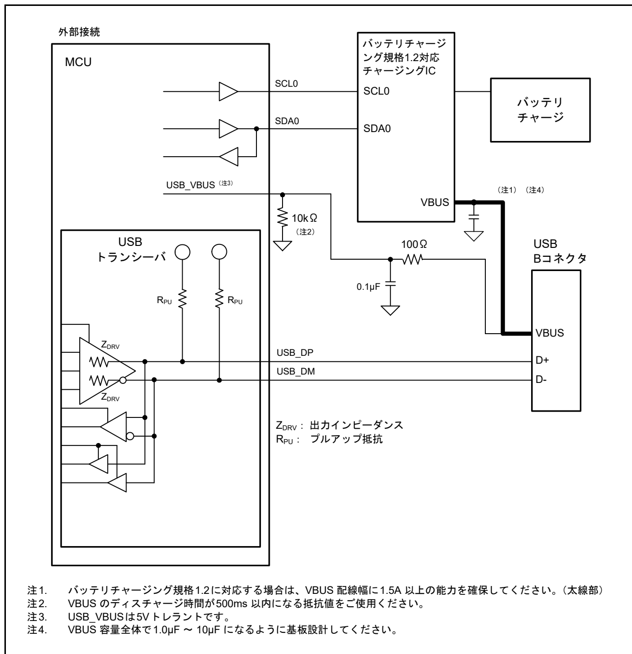
図 26.8 バッテリチャージング規格 1.2 対応 USB コネクタのファンクション接続例
