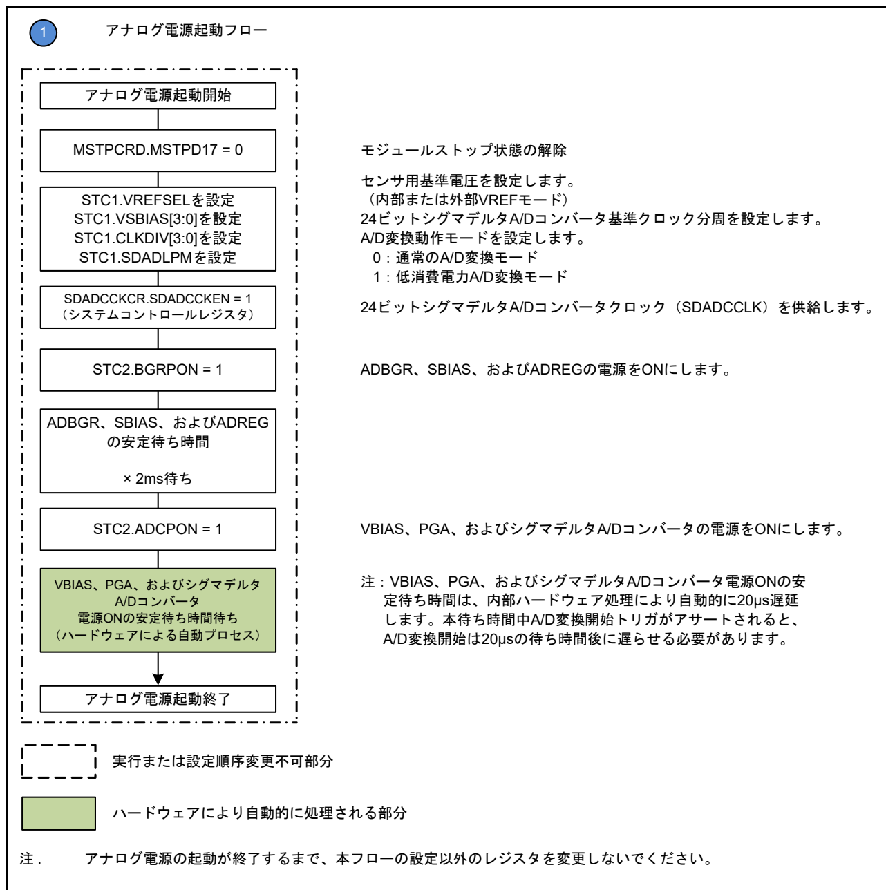
図 33.23 アナログ電源起動フロー
