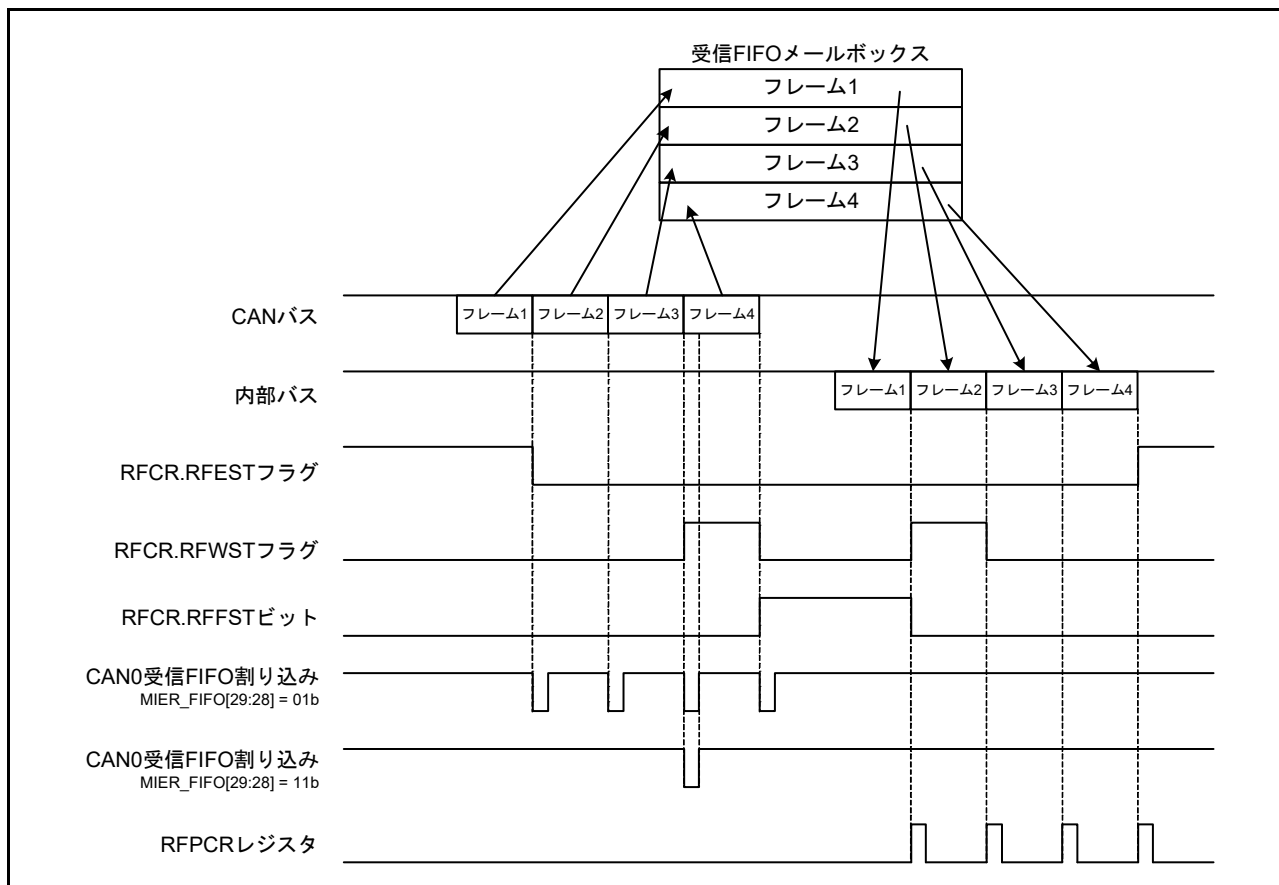
図 29.2 受信 FIFO メールボックスの動作（MIER_FIFO レジスタのビット 29、28 が 01b または 11b のとき）
