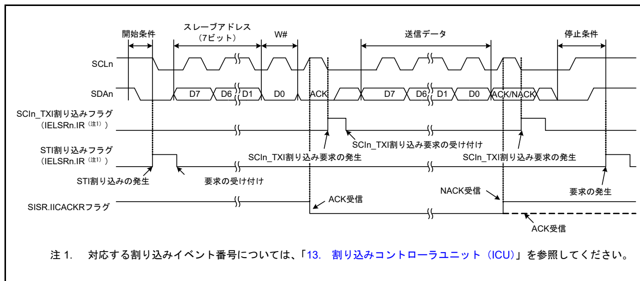
図 27.64 簡易 IIC モードのマスタ送信の動作例 1 (7 ビットスレーブアドレス、送信割り込み、受信割り込み使用時)
