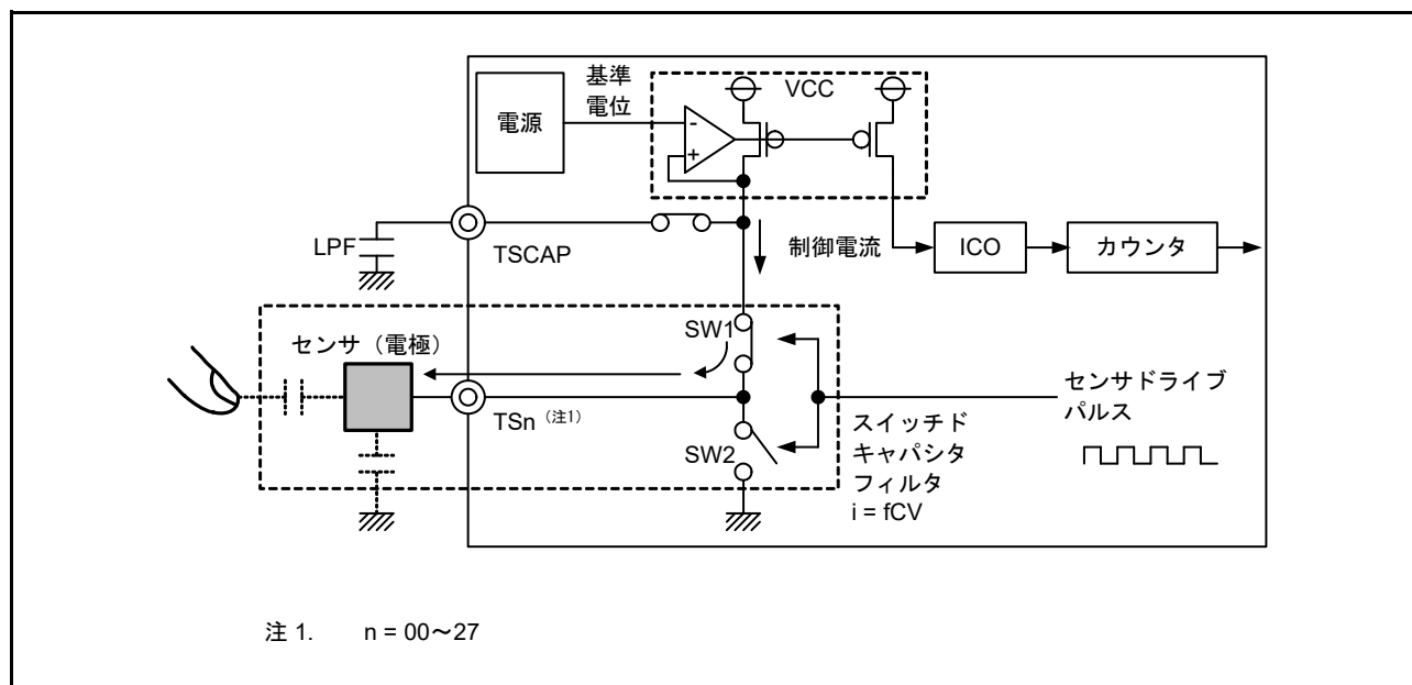
図 40.5 充電動作
