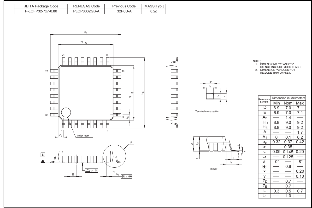
図 2.2 LQFP 32 ピン
