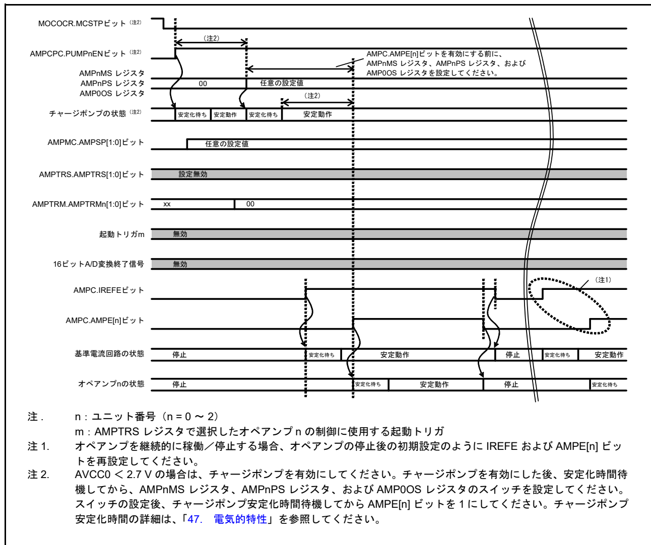
図 37.6 オペアンプの制御動作 (ソフトウェアトリガモードによる制御) (ソフトウェアトリガモードによって基準電流回路およびオペアンプを起動/停止する場合)
