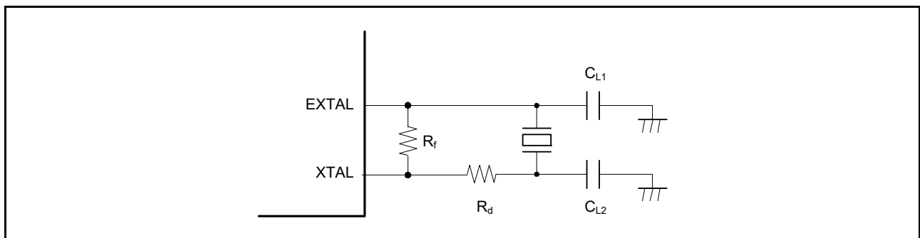
図 9.4 水晶振動子の接続例
