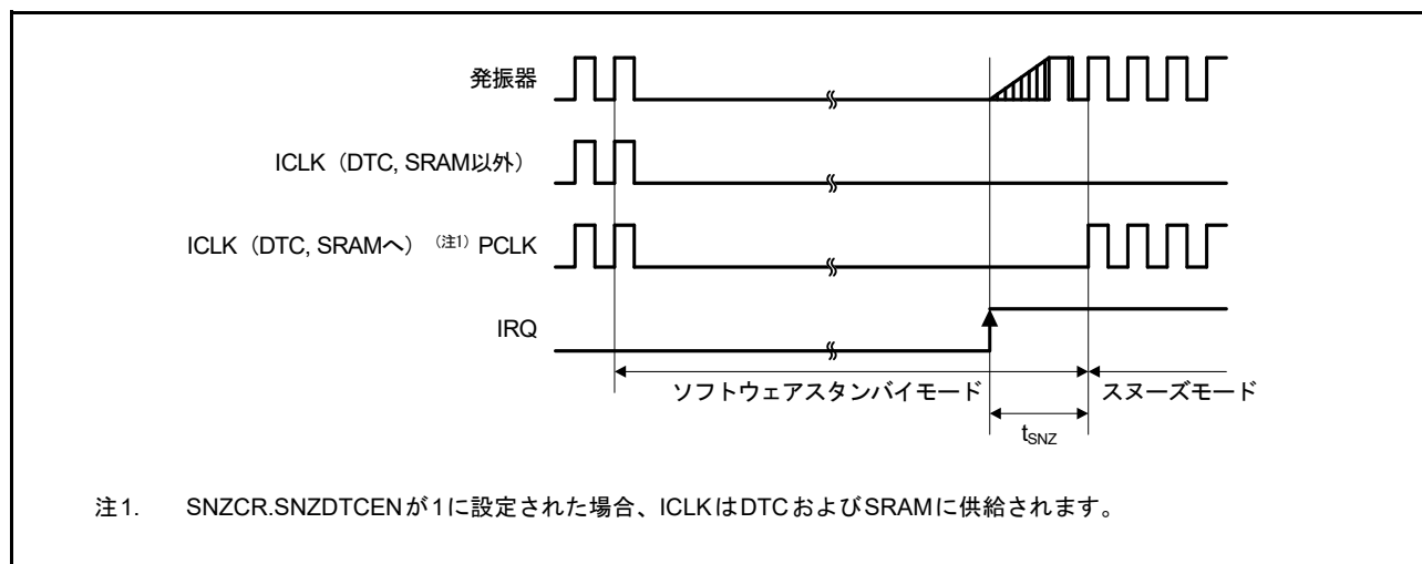
図 47.33 ソフトウェアスタンバイモードからスリープモードへの復帰タイミング
