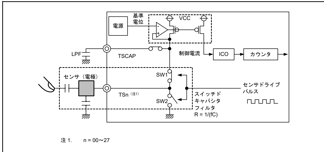
図 40.4 計測部回路
