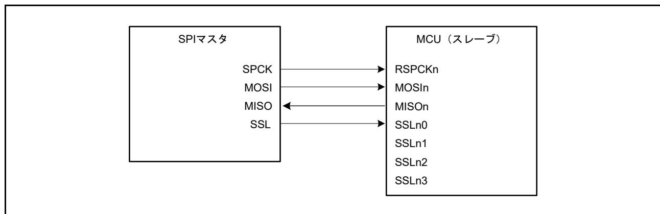
図 30.6 シングルマスタとシングルスレーブの構成例 (MCU はスレーブ、CPHA = 0)
