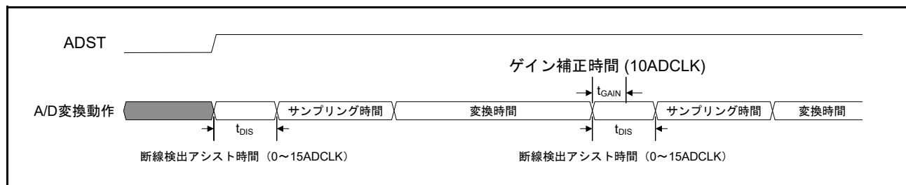
図 32.30 断線検出アシスト機能を使用した場合の A/D 変換動作図
