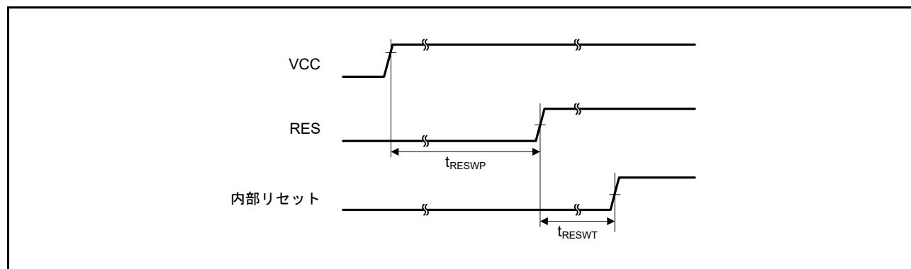
図 47.29 電源投入時リセット入力タイミグ
