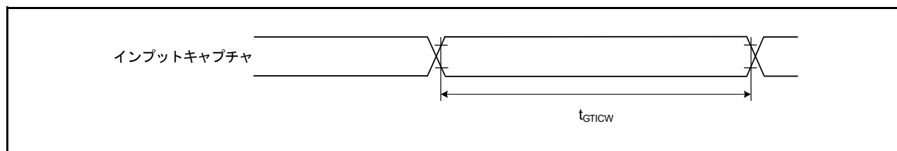
図 47.38 GPT インプットキャプチャタイミング
