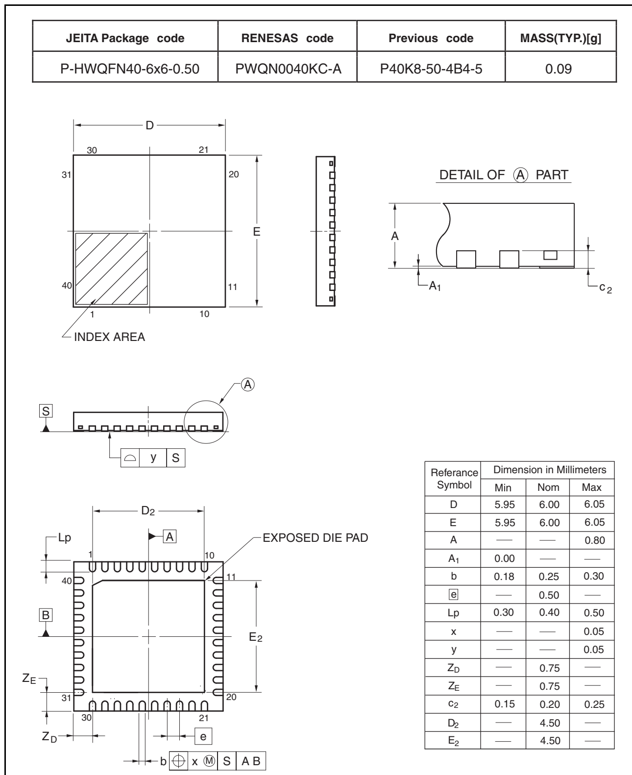
図 2.5 QFN 40 ピン
