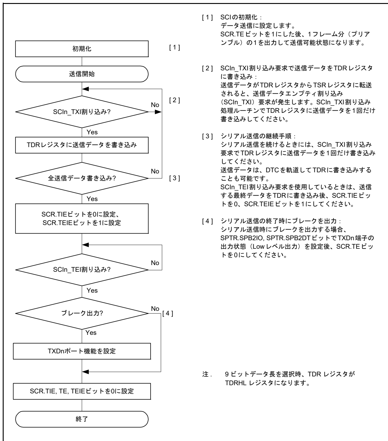
図 27.12 調歩同期式モードにおけるシリアル送信のフローチャート例（非 FIFO 選択時）
