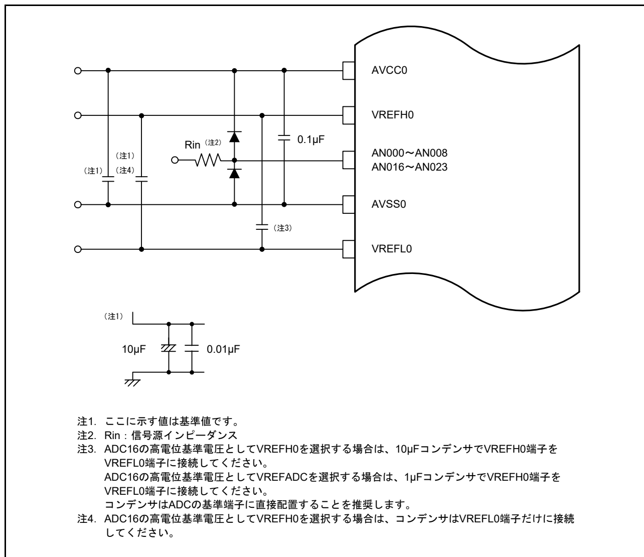
図 32.39 アナログ入力用保護回路例
