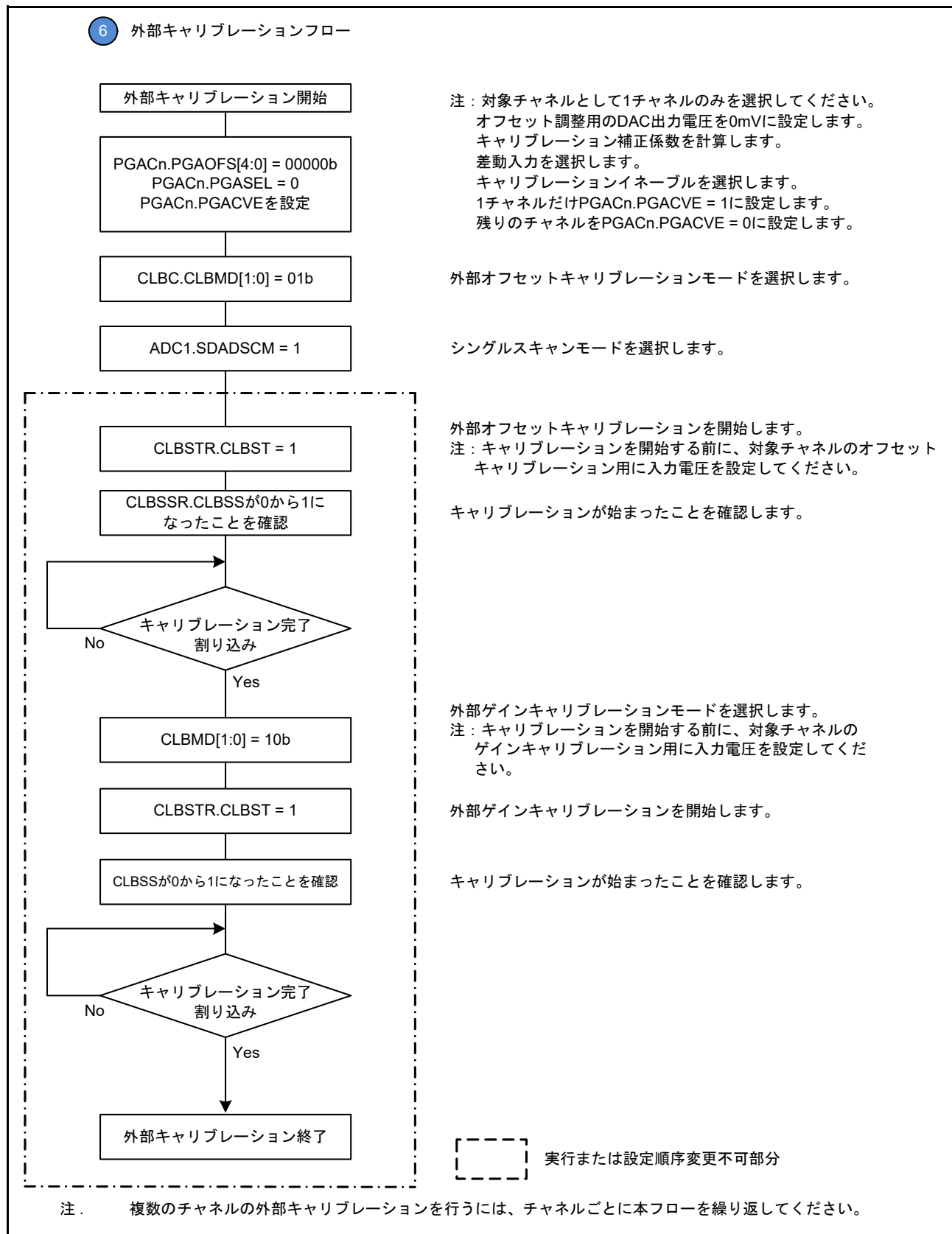
図 33.28 外部キャリブレーションフロー
