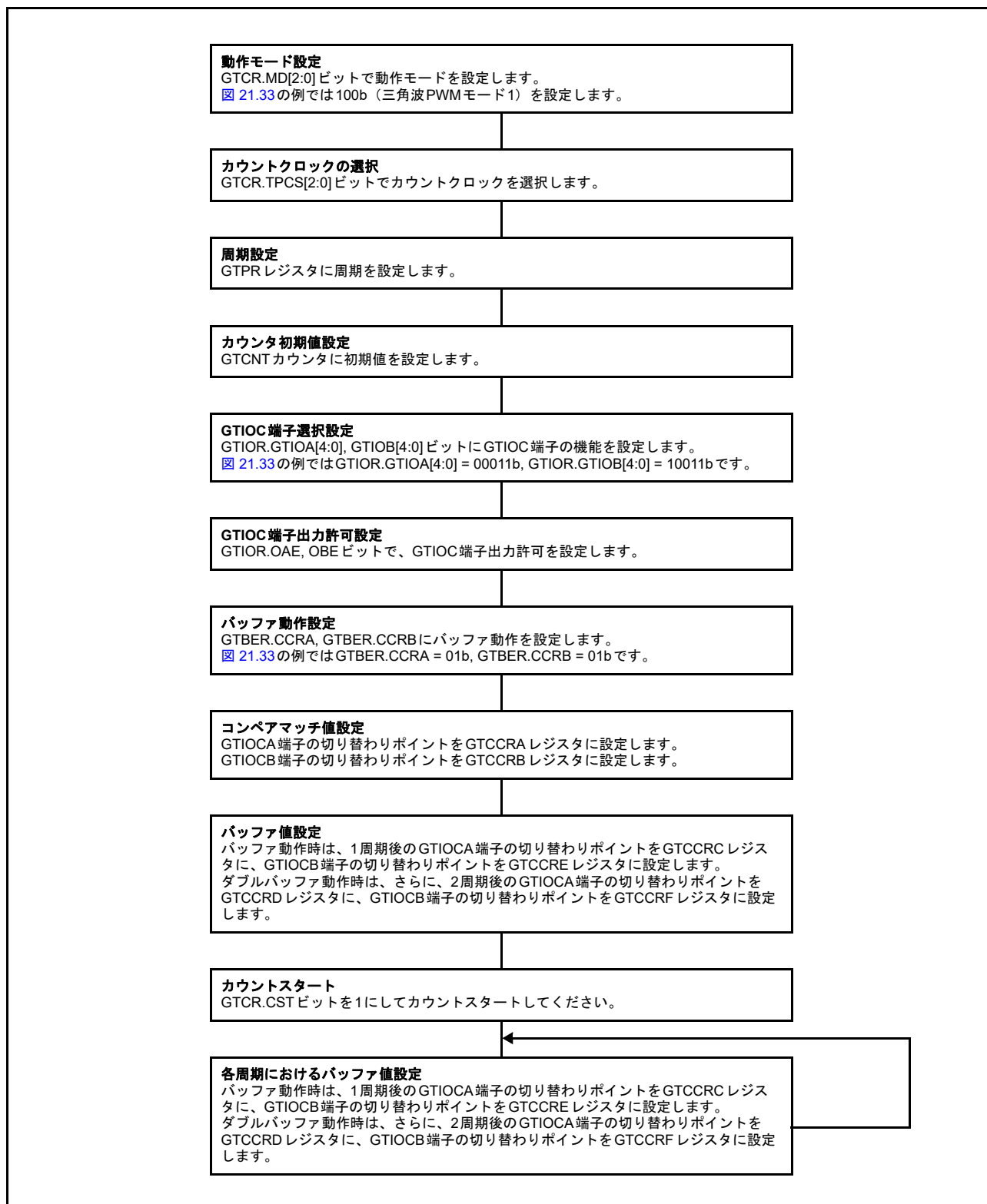
図 21.34 三角波 PWM モード 1 設定例
