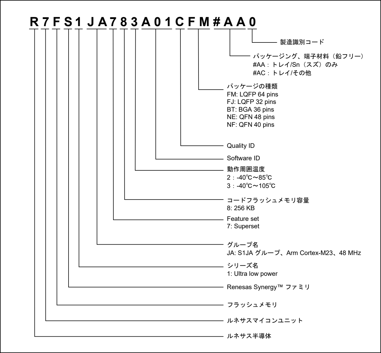
図 1.2 型名の読み方
