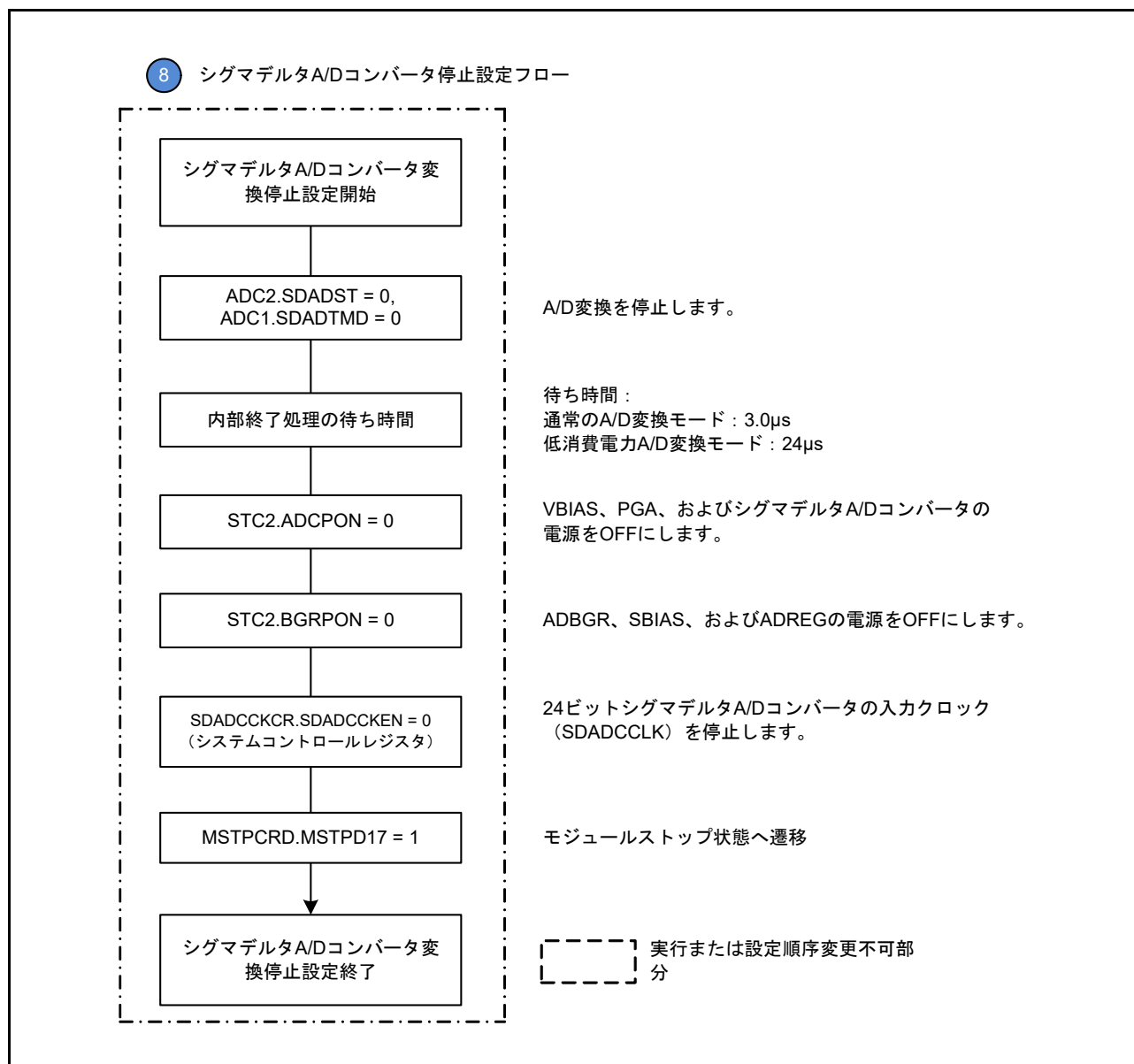
図 33.30 SDADC24 停止設定フロー
