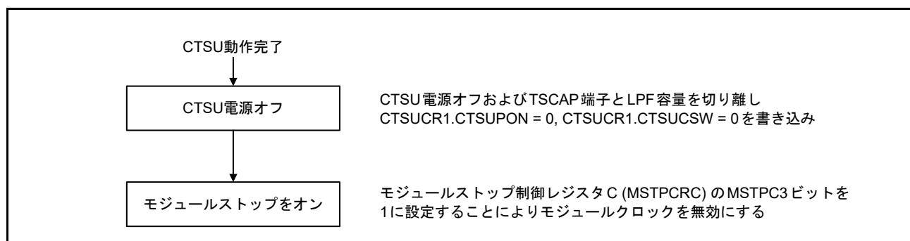
図 40.10 CTSU 停止フロー
