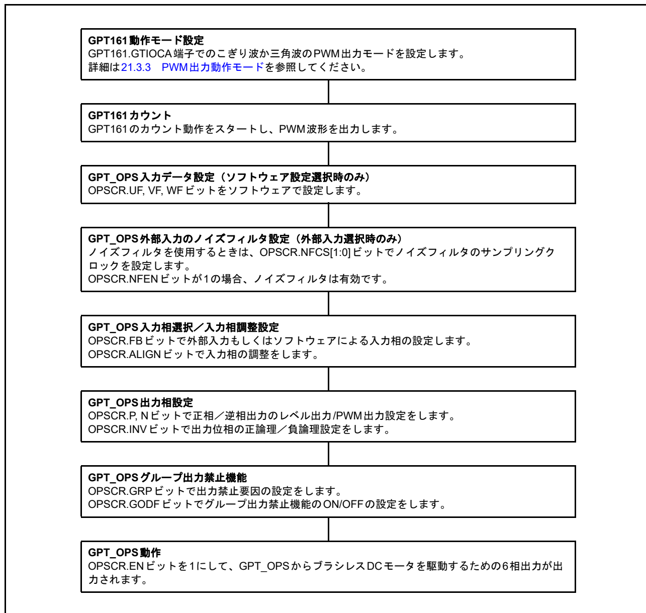
図 21.81 GPT_OPS スタート動作設定例
