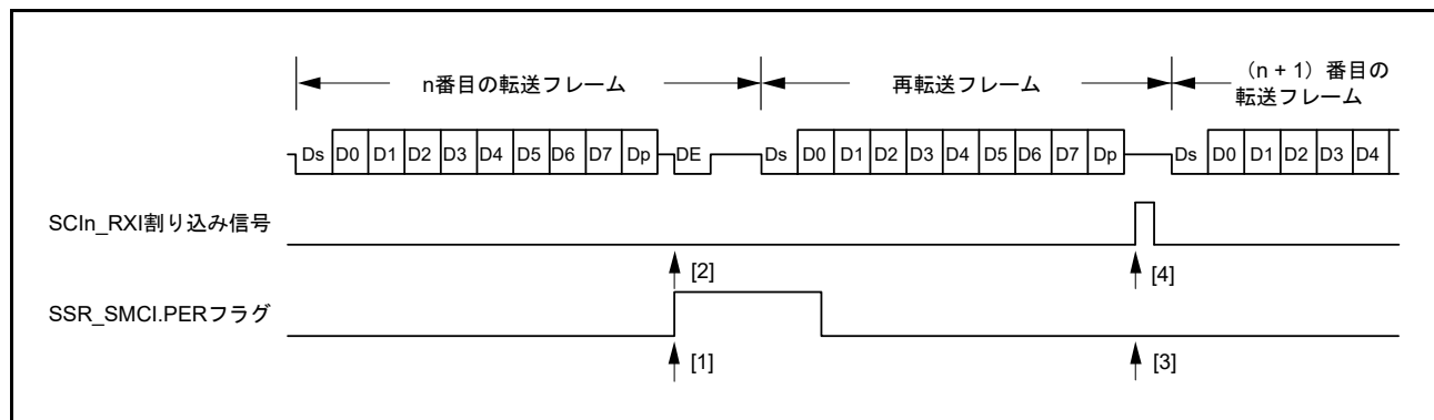
図 27.55 SCI 受信モードでの再転送動作（受信時の再転送動作）
