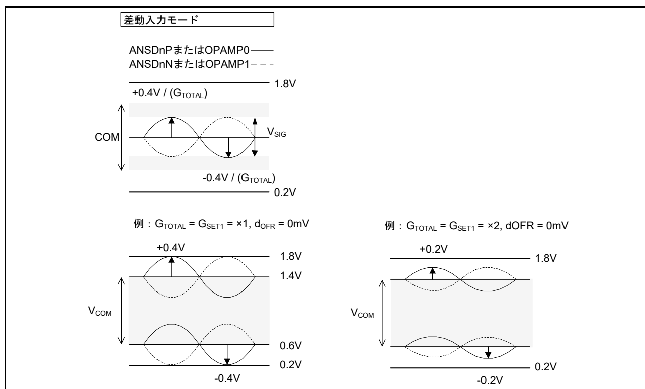
図 33.8 差動入力モード時の入力電圧範囲
