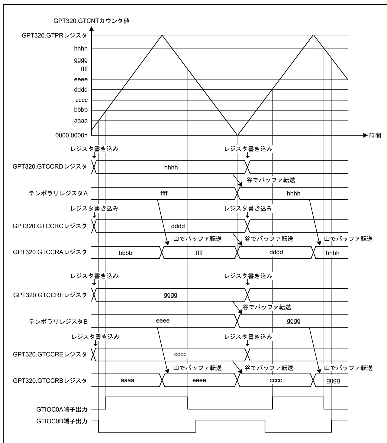
図 21.37 三角波 PWM モード 3 動作例 (カウントスタート時に GTIOC0A 端子 = Low 出力 / GTIOC0B 端子 = High 出力、GTCRA/GTCRB レジスタのコンペアマッチ時にトグル出力、周期の終わりで出力保持の場合)
