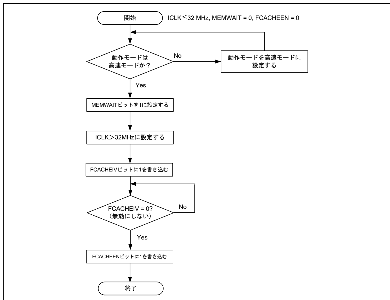
図 9.2 ICLK > 32MHz に設定する場合
