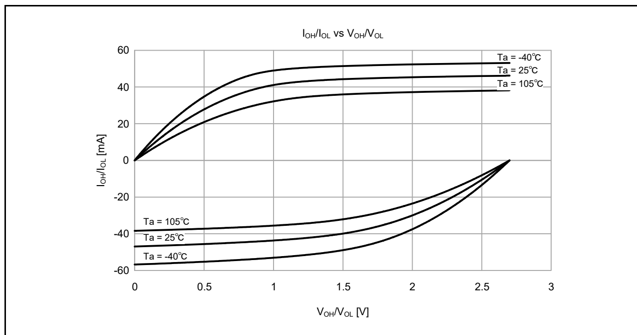
図 47.13 中駆動出力選択時の V_{CC} = 2.7\text{ V} での V_{OH}/V_{OL} および I_{OH}/I_{OL} 温度特性（参考データ）
