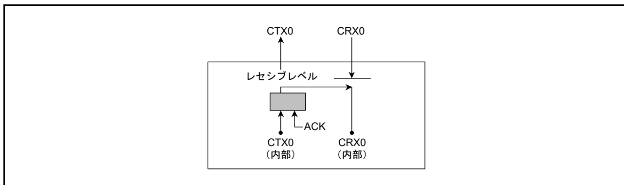
図 29.8 セルフテストモード 1 選択時の接続
