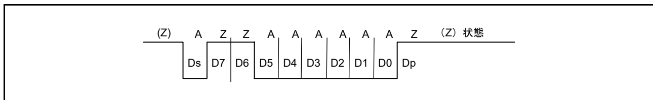
図 27.48 インバースコンベンション (SCMR.SDIR ビット = 1、SCMR.SINV ビット = 1、SMR_SMCI.PM ビット = 1)
