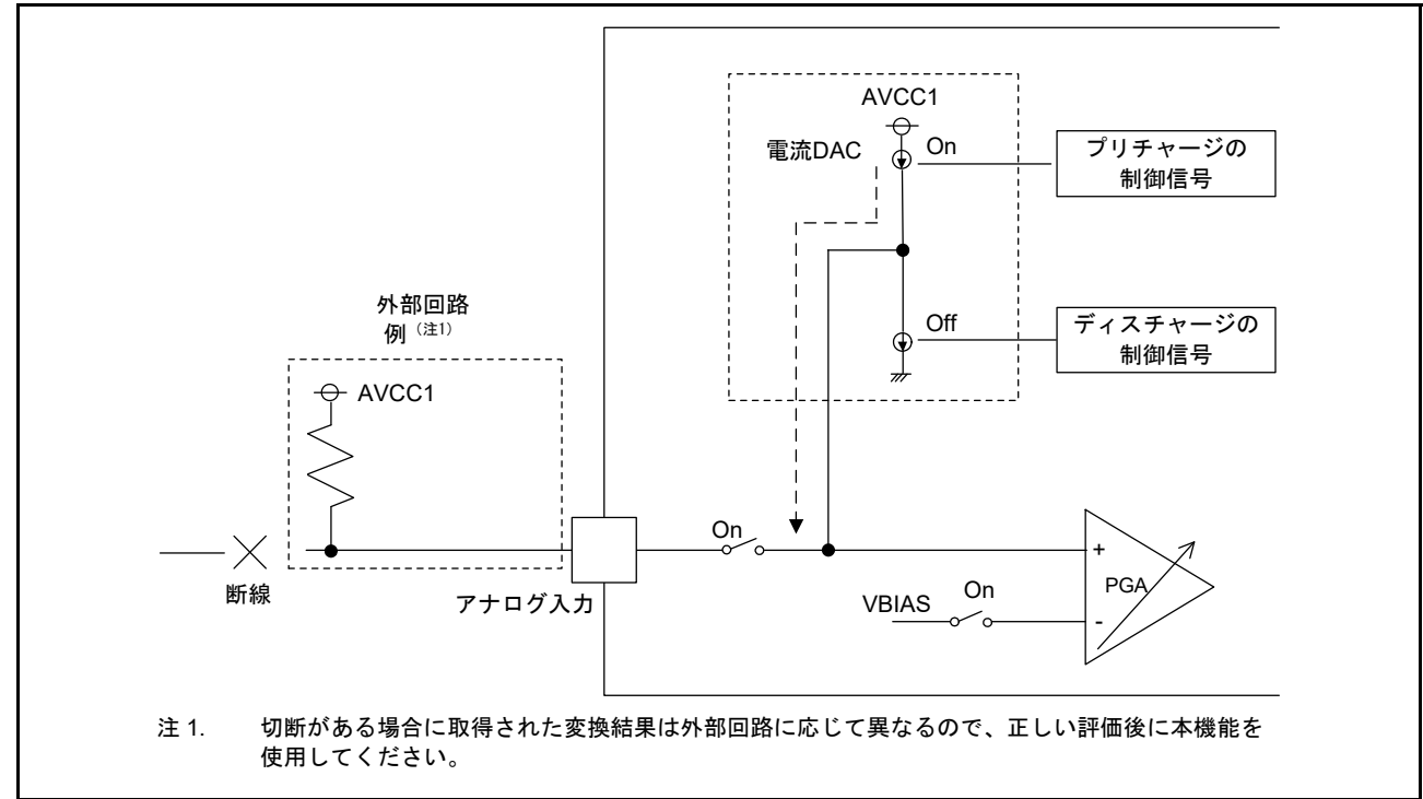
図 33.19 シングルエンド入力モード（正側）でプリチャージ選択時の切断検出例
