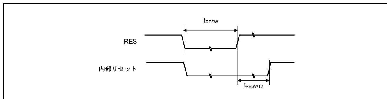
図 47.30 リセット入力タイミグ (1)
