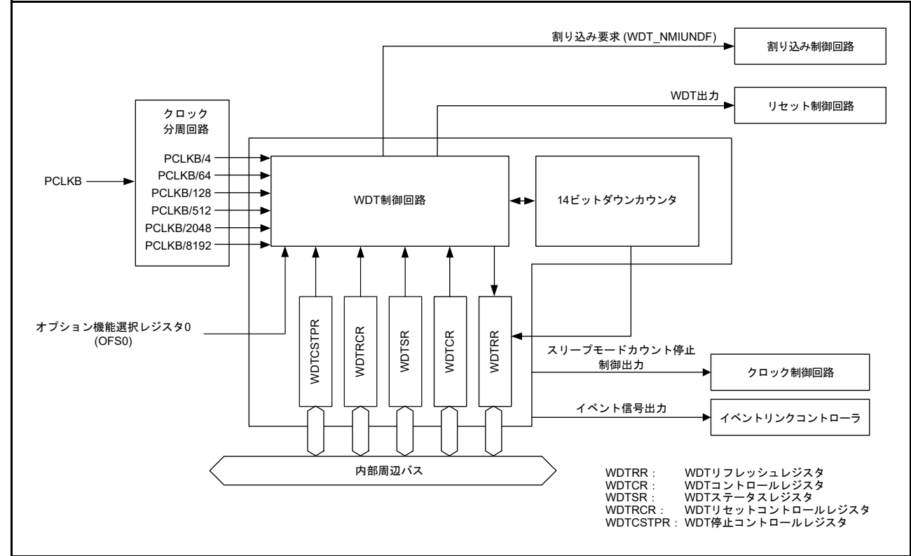
図 24.1 WDT のブロック図
