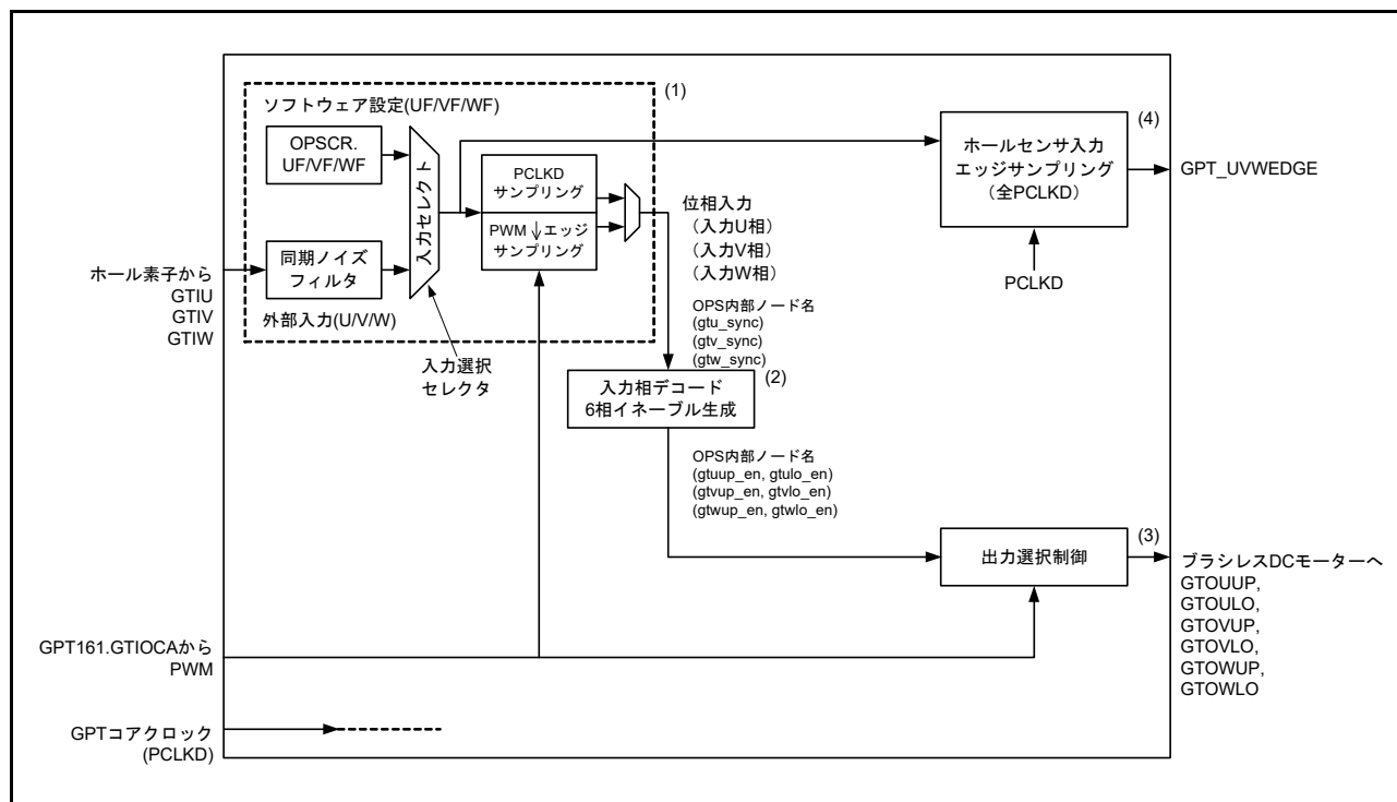
図 21.77 GPT_OPS 制御フロー概念図
