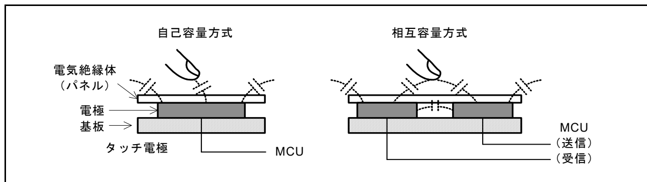
図 40.2 自己容量方式と相互容量方式
