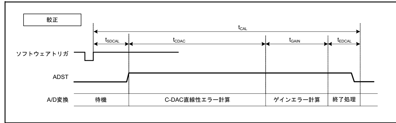
図 32.36 キャリブレーションタイミング
