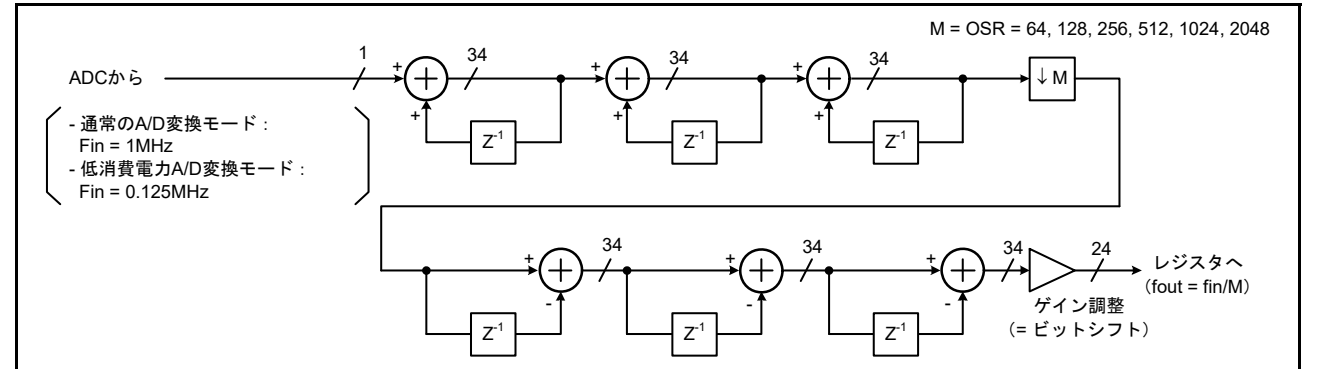
図 33.17 デジタルフィルタのブロック図
