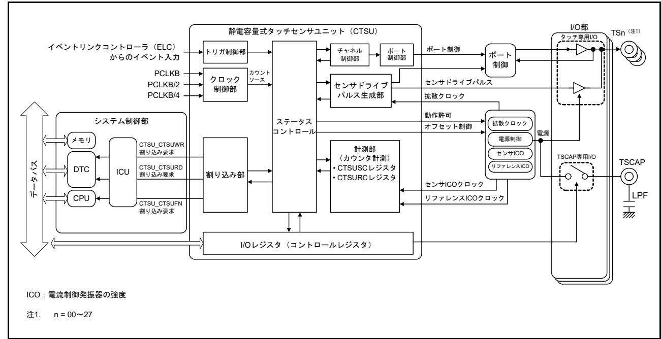
図 40.3 CTSU のブロック図
