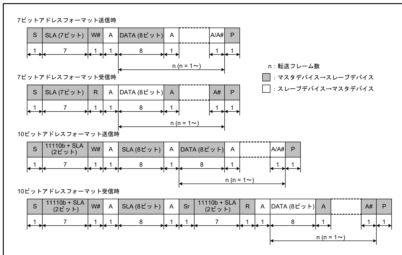
図 27.58 I 2 C バスフォーマット
