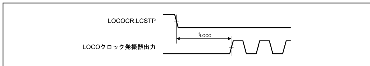
図 47.26 LOCO クロック発振開始タイミング
