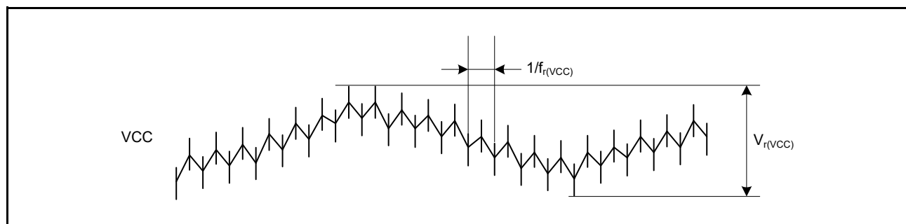
図 47.24 リップル波形
