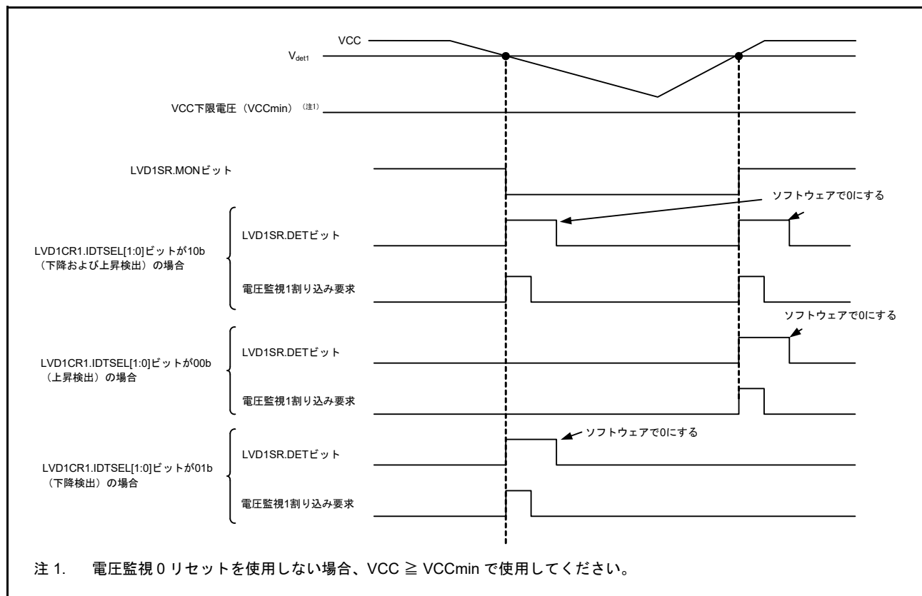
図 8.5 電圧監視 1 割り込みの動作例
