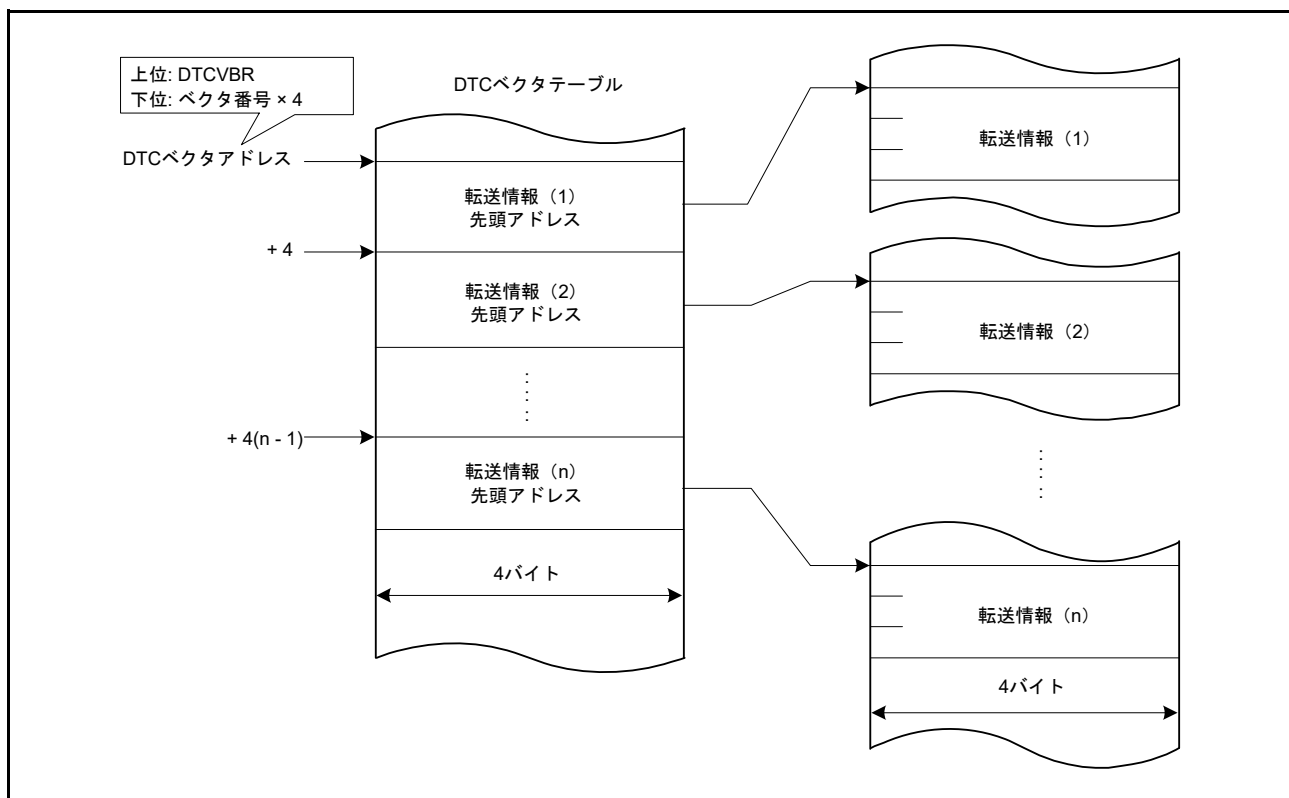
図 16.2 DTC ベクタテーブルと転送情報の対応
