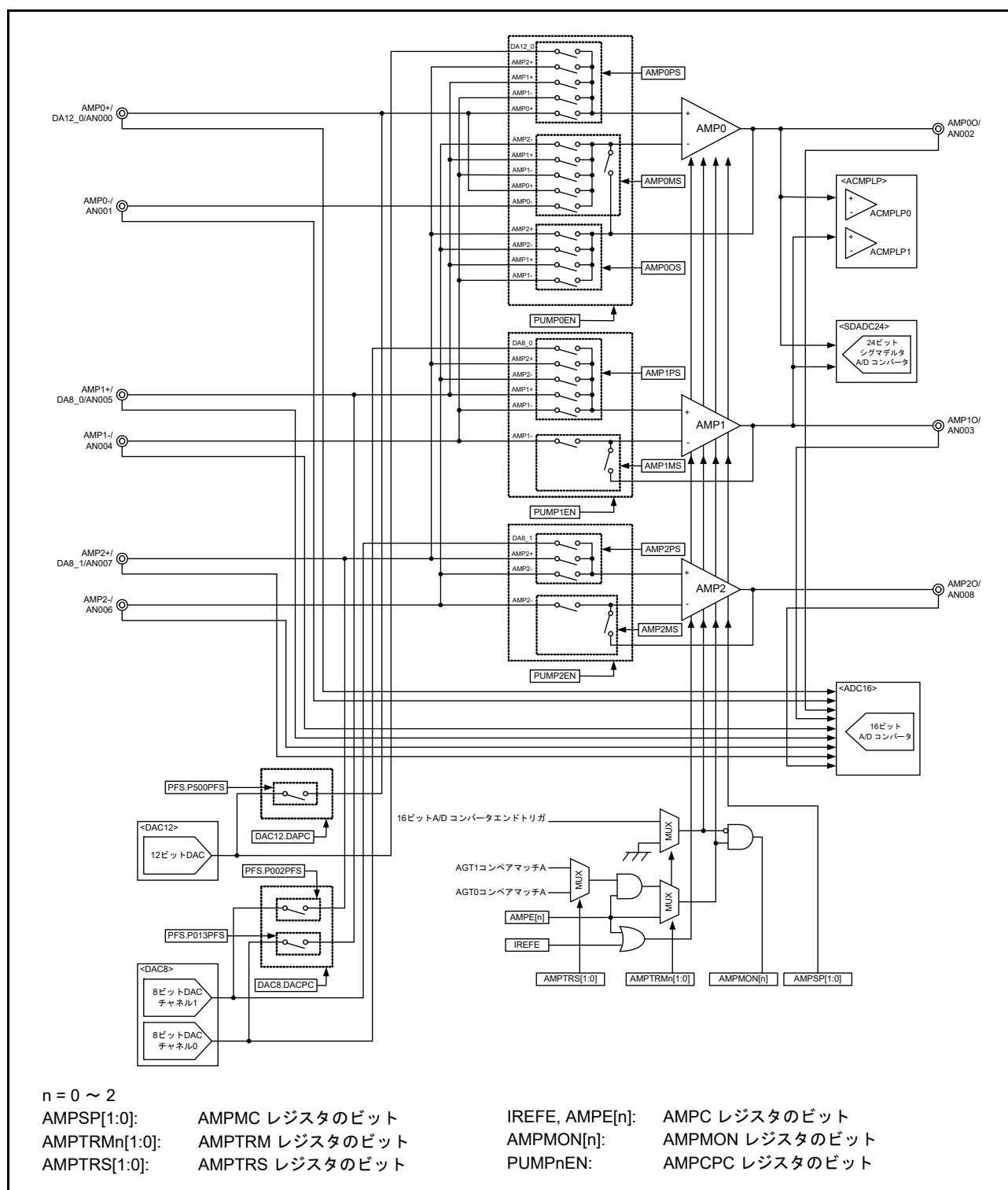
図 37.1 オペアンプのブロック図
