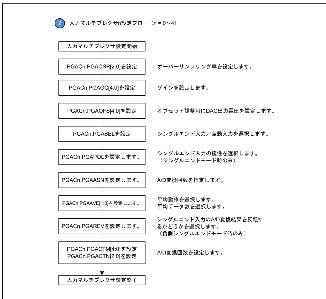
図 33.24 入力マルチプレクサ設定フロー
