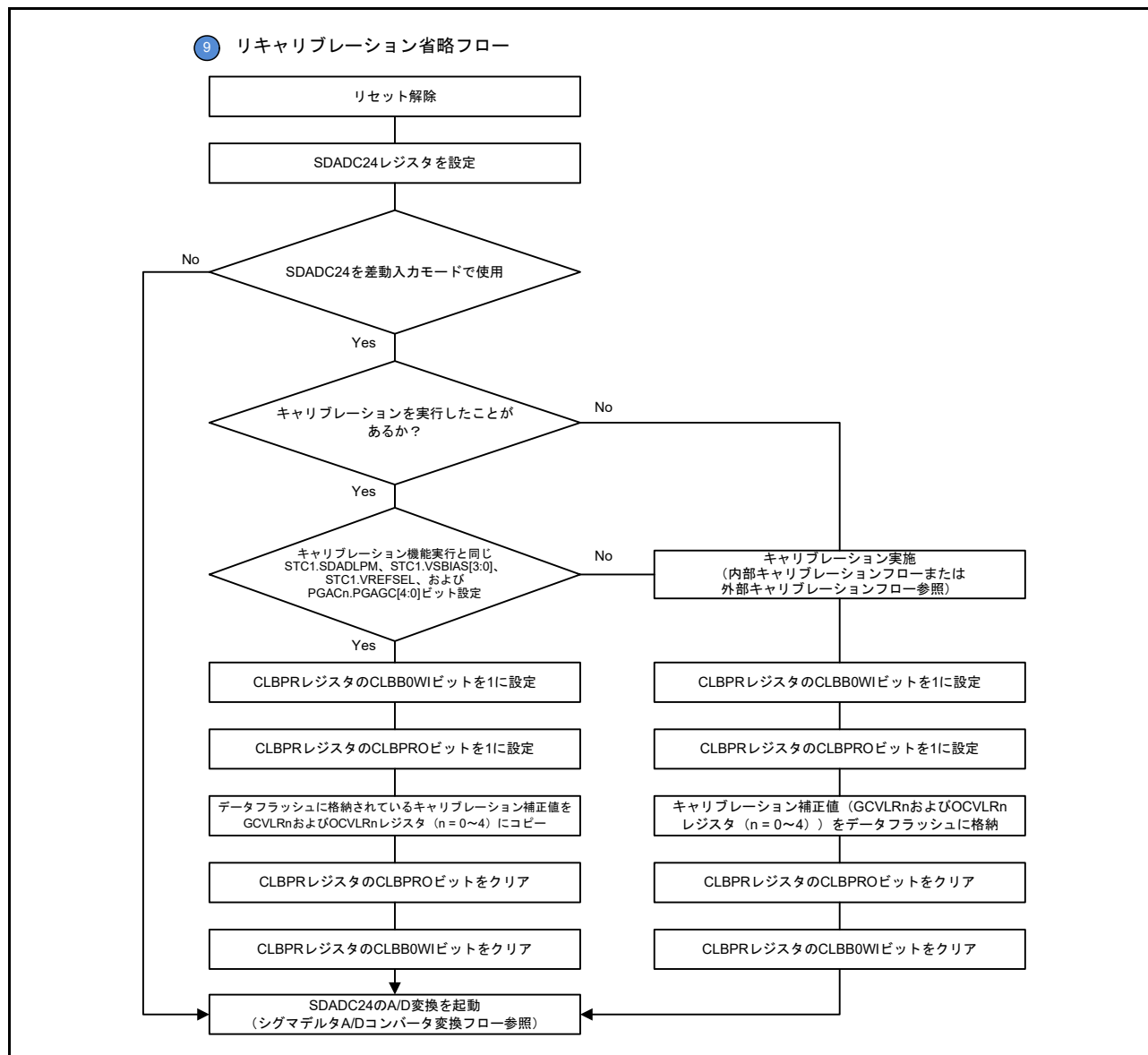
図 33.31 リキャリブレーション省略フロー
