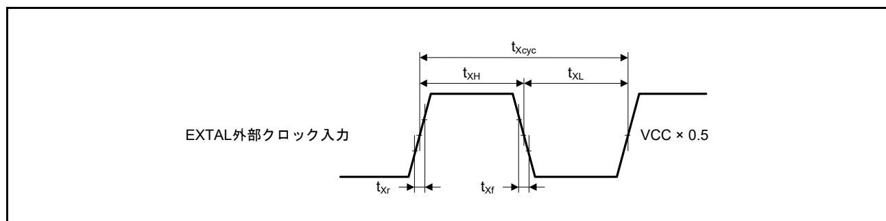
図 47.25 EXTERNAL 外部クロック入力タイミング
