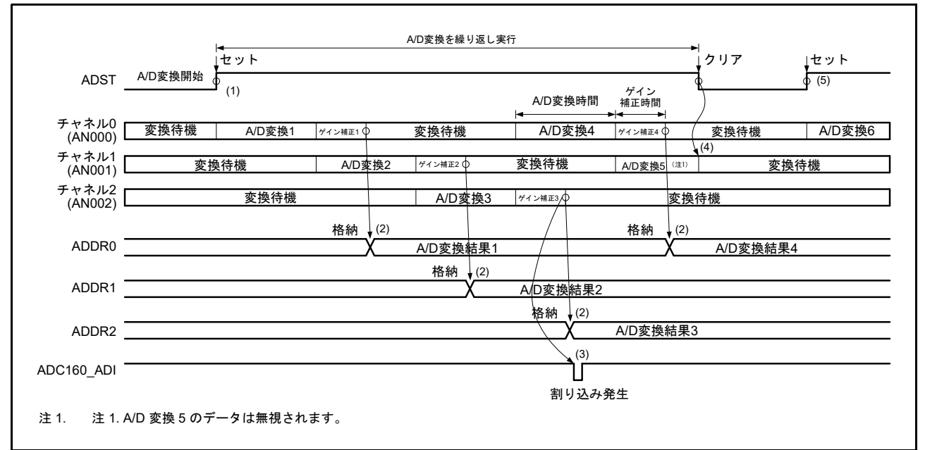
図 32.15 連続スキャンモードの基本動作例 (AN000 ~ AN002 選択)
