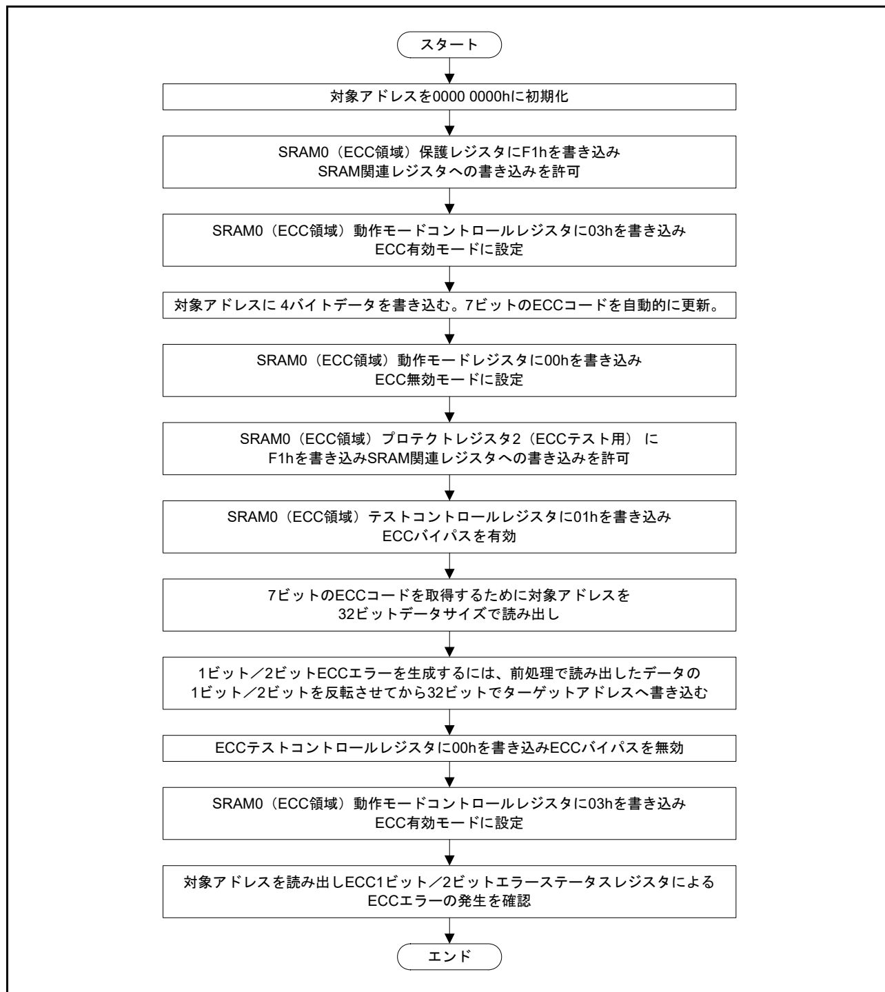
図 42.1 ECC デコーダのテスト方法
