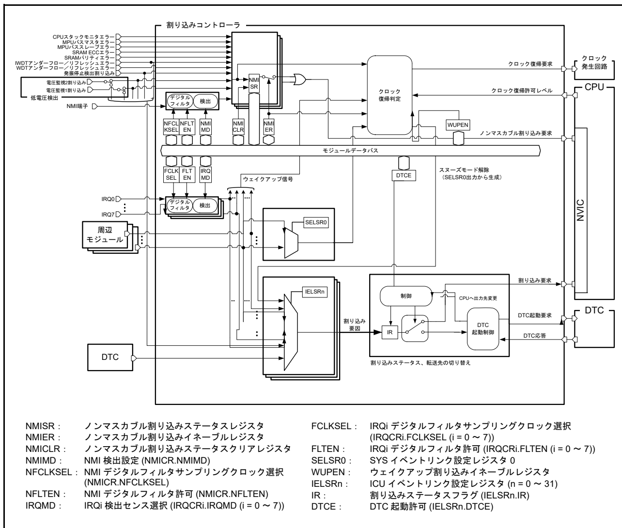
図 13.1 ICU のブロック図
