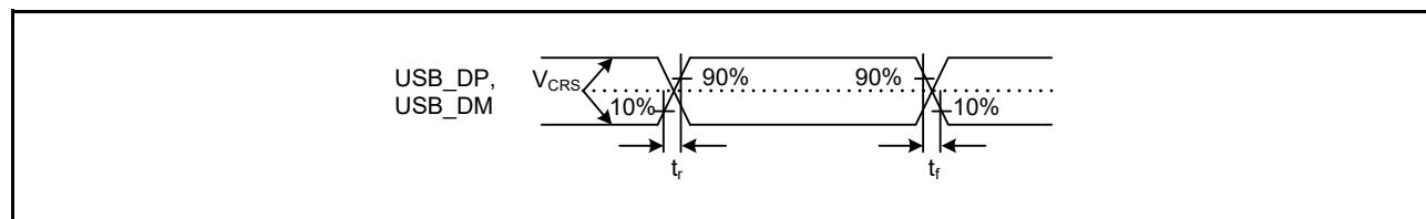
図 47.59 USB_DP および USB_DM 出力タイミング
