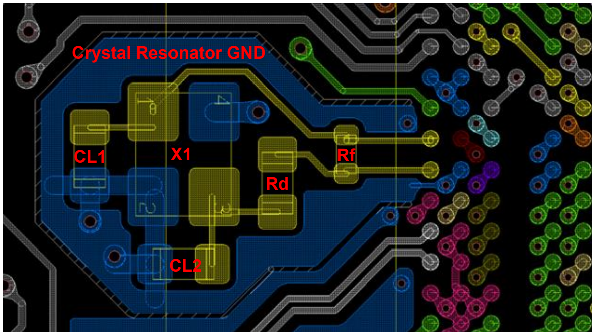
図 3.3 基板の 1 層目 (Layer1) のレイアウト例
