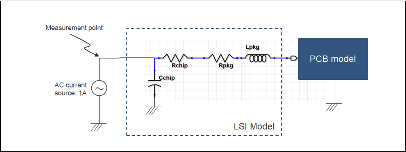
図 10.4 トポロジー
