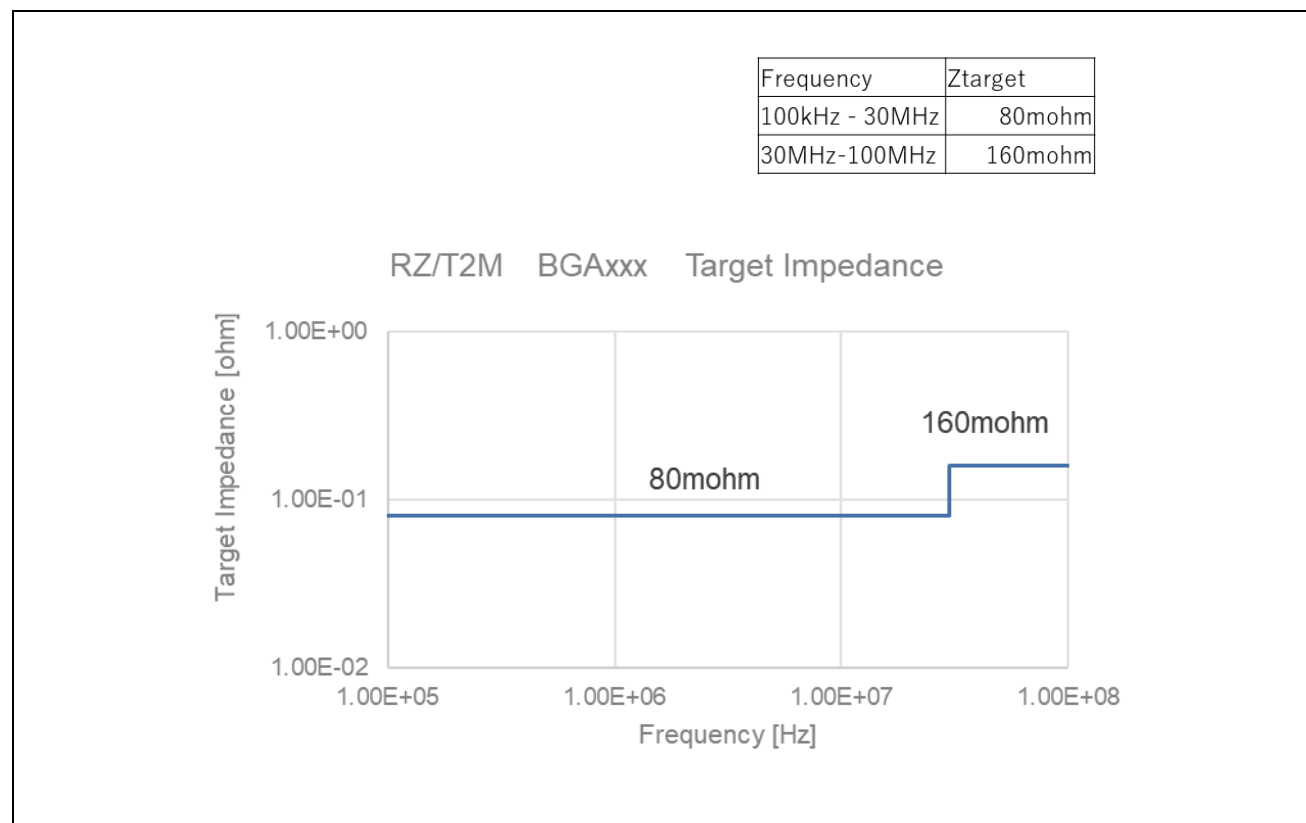
図 10.2 VDD ターゲットインピーダンス (320-FBGA / 225-FBGA)
