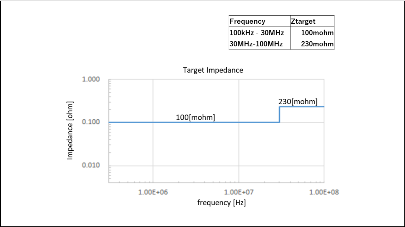
図 10.7 VDD ターゲットインピーダンス (196-FBGA)
