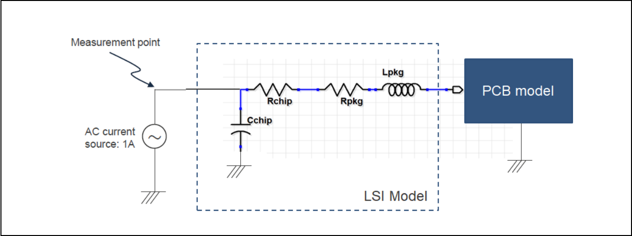
図 10.6 トポロジー
