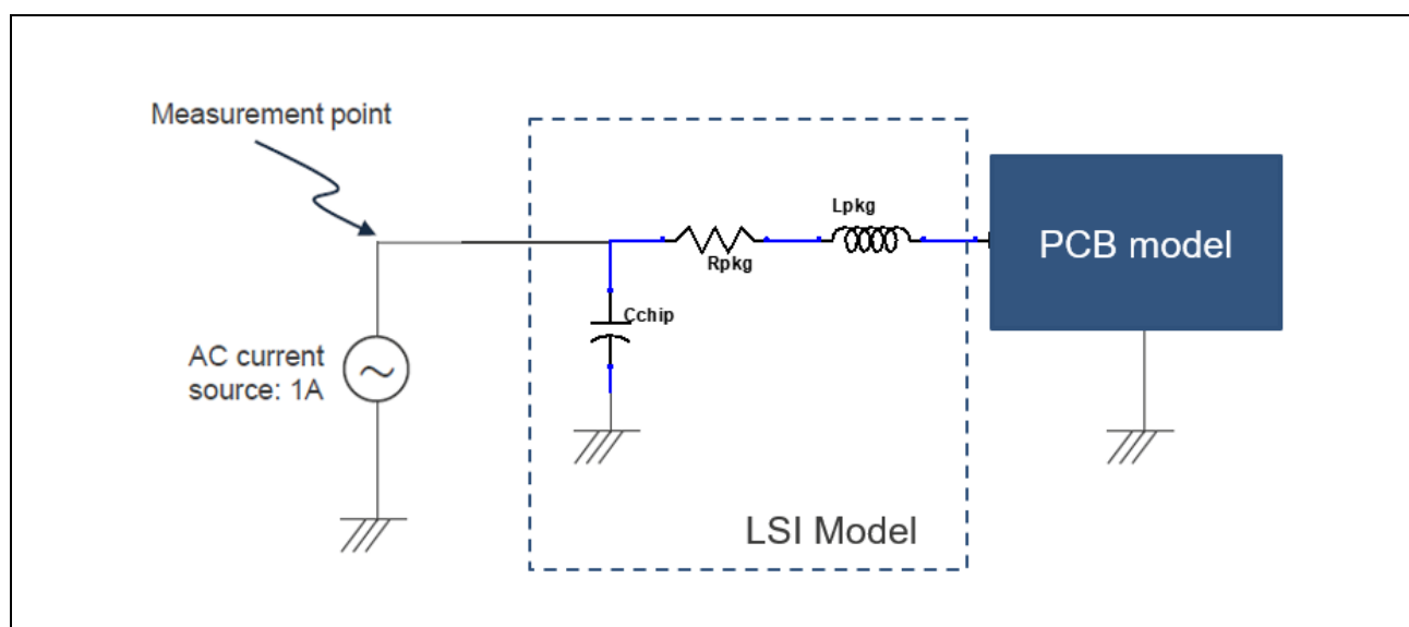
図 10.1 トポロジー
