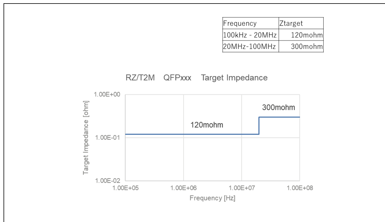
図 10.3 VDD ターゲットインピーダンス (176-LQFP / 128-LQFP )
