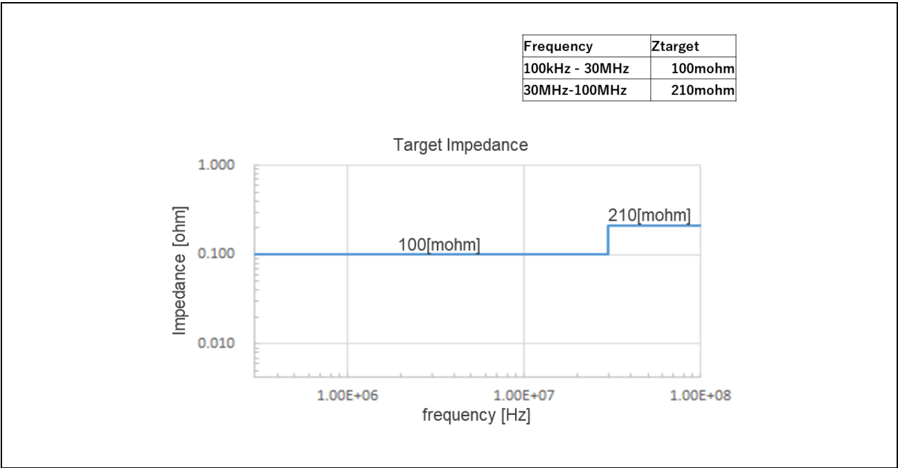
図 10.5 VDD ターゲットインピーダンス (121-FBGA / 225-FBGA)
