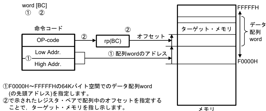
図3 - 30 word[BC]の例
