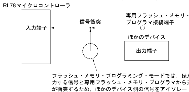
図30-5 信号の衝突 (RESET 端子)
