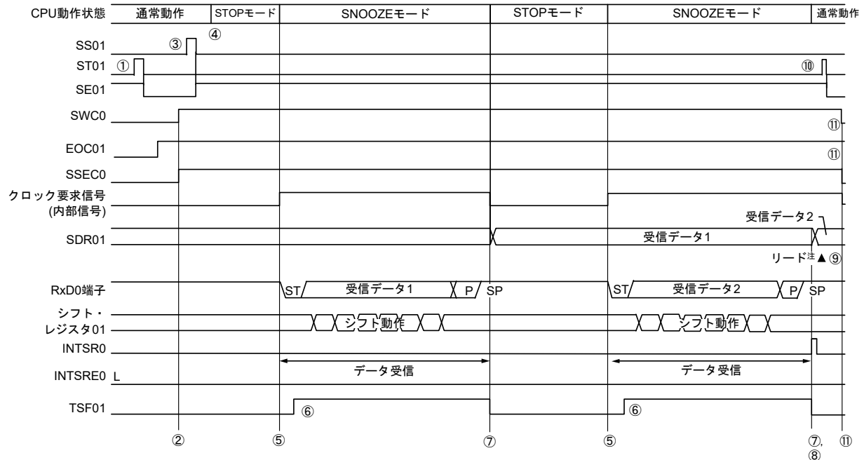
図15 - 98 SNOOZEモード動作(EOCm1 = 1, SSECm = 1)時のタイミング・チャート
