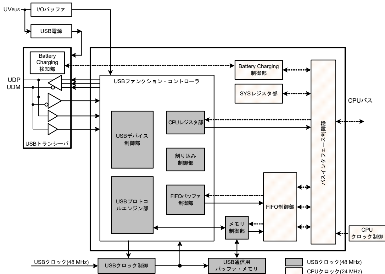
図17-1 USBモジュールのブロック図
