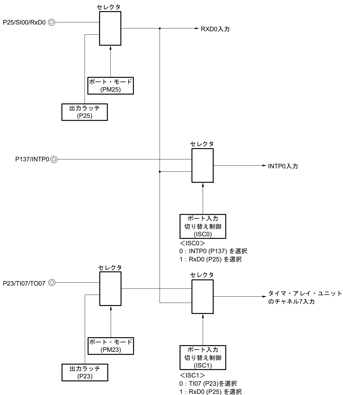
図15 - 107 LINの受信操作のポート構成図
