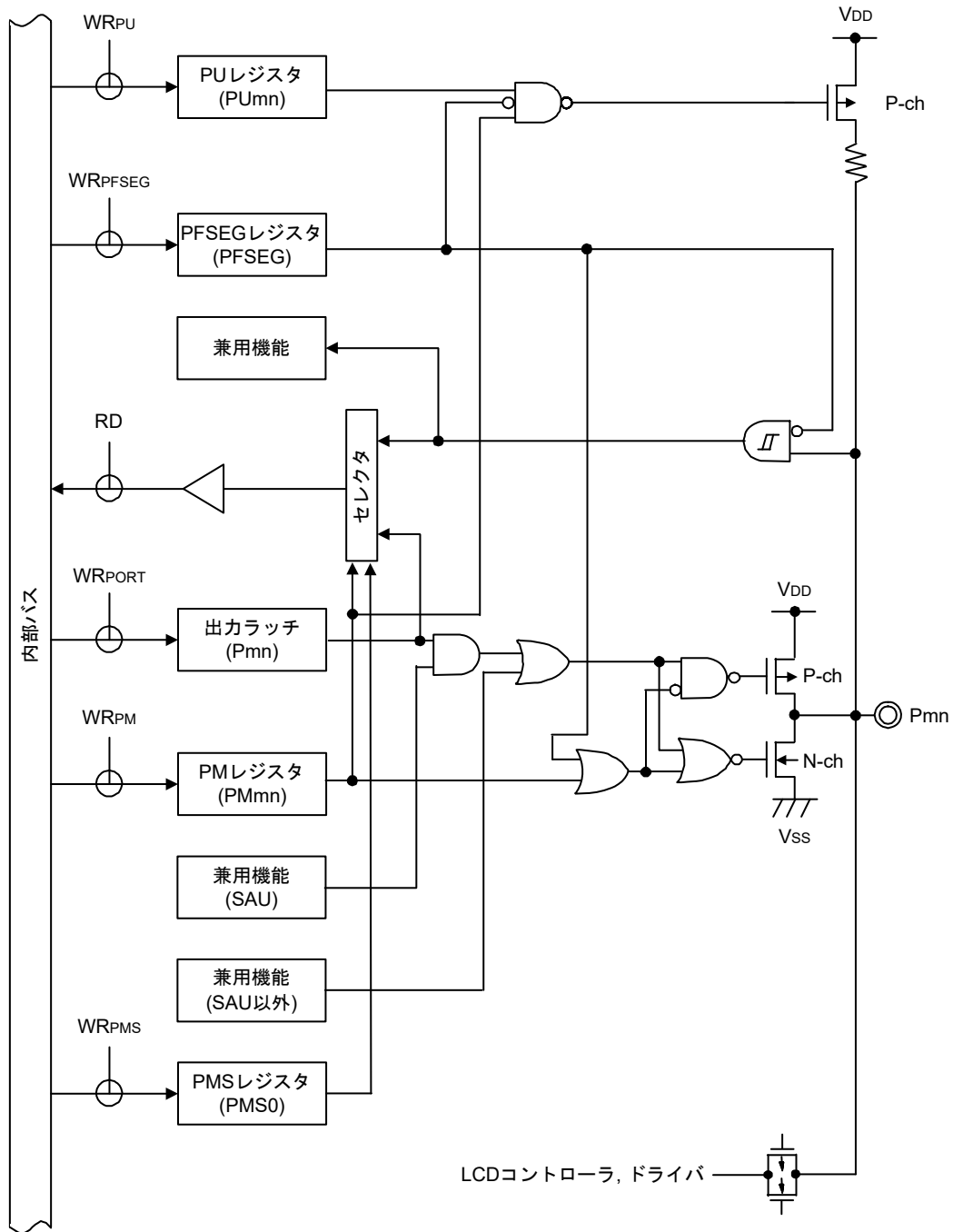
図2-9 端子タイプ7-5-4の端子ブロック図
