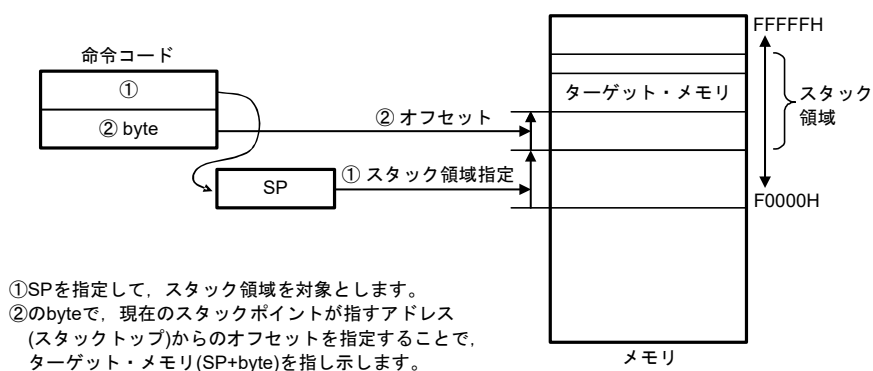
図3 - 27 [SP+byte]の例
