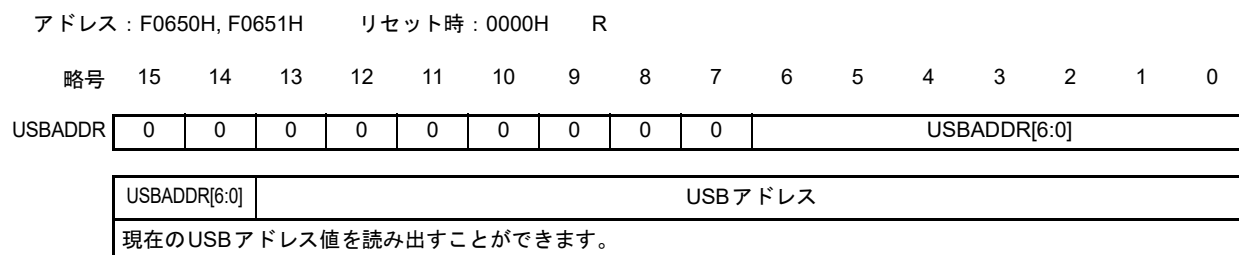
図 17-25 USBアドレス・レジスタ (USBADDR) のフォーマット
