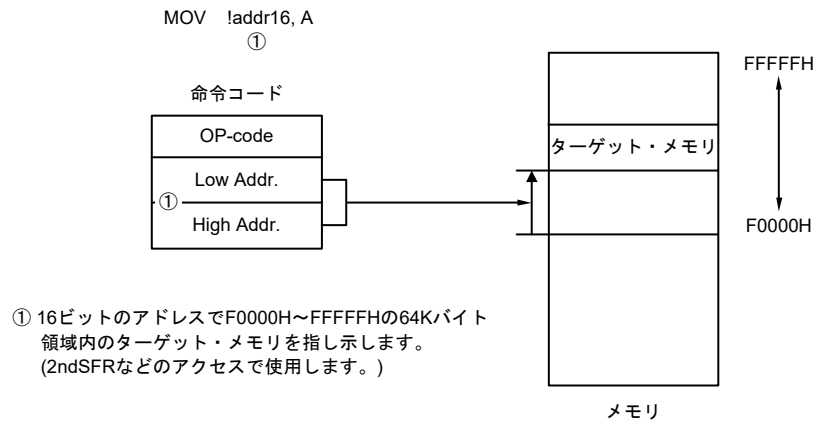
図3 - 21 !addr16の例
