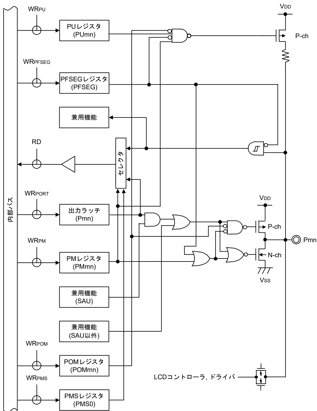
図2-12 端子タイプ7-5-10の端子ブロック図
