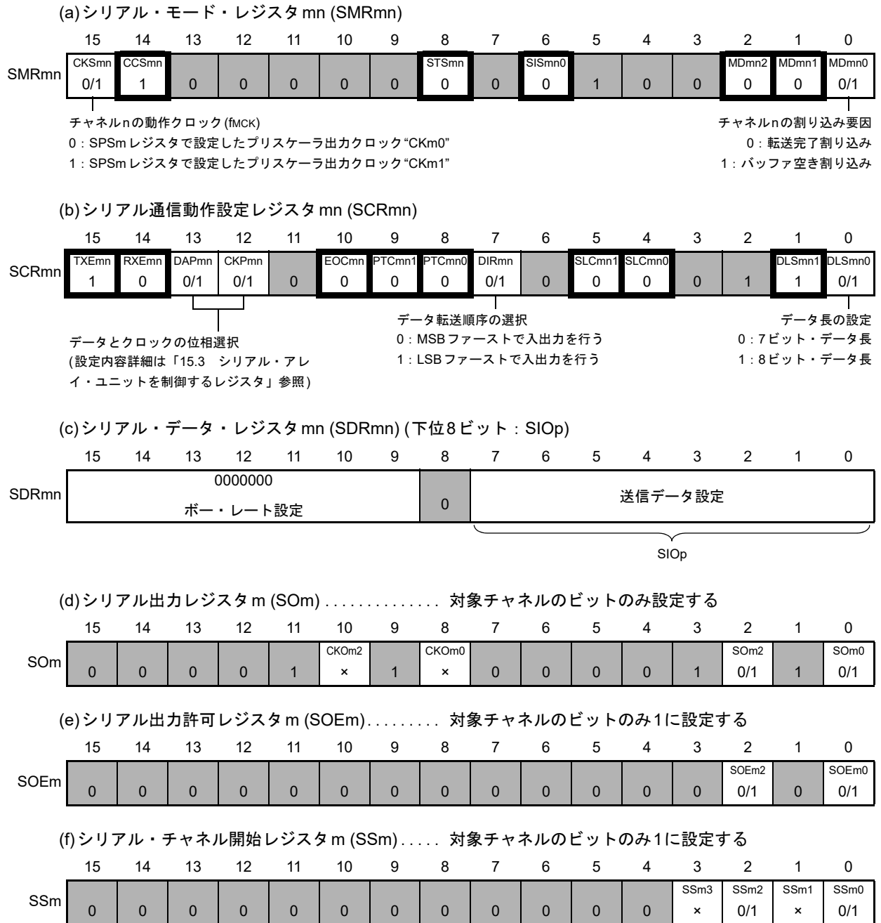
図 15 - 52 簡易SPI (CSI00, CSI10, CSI20, CSI30)のスレーブ送信時のレジスタ設定内容例
