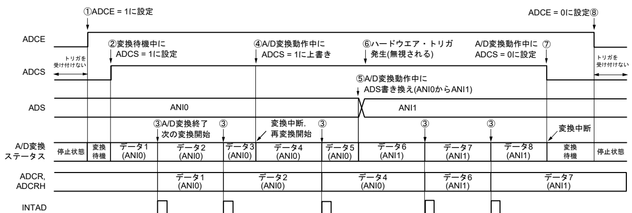
図12-18 ソフトウェア・トリガ・モード(セレクト・モード, 連続変換モード)動作タイミング例
