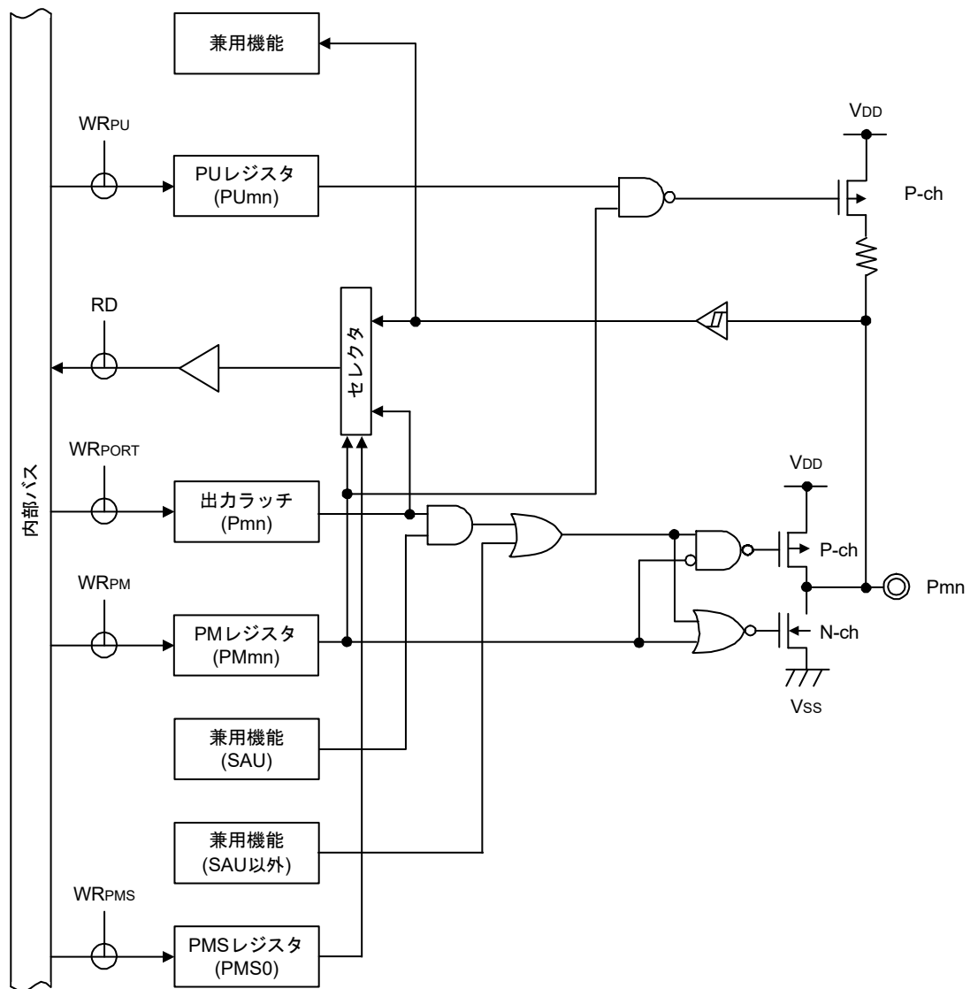
図2-6 端子タイプ7-1-3の端子ブロック図
