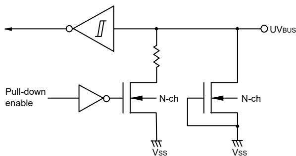
図2 - 17 端子タイプ17-11-1の端子ブロック図
