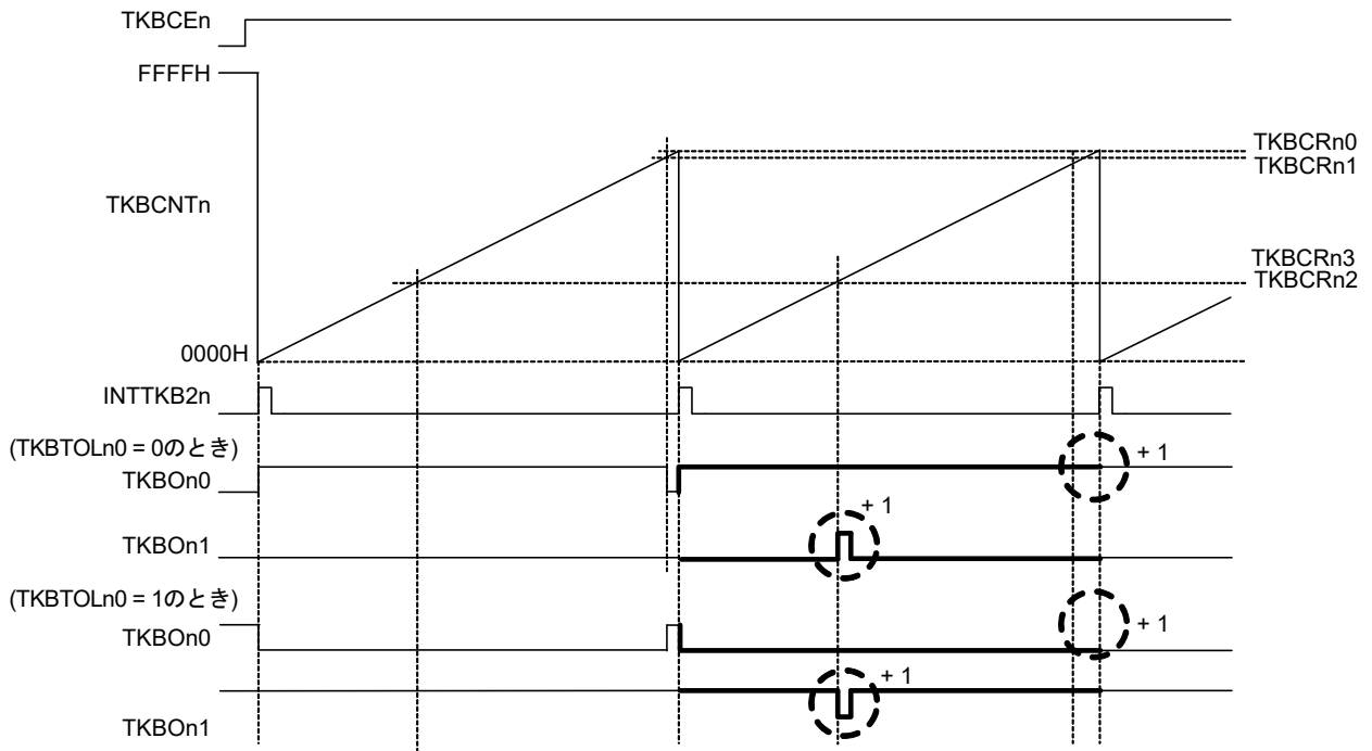
図7-76 ディザリング動作の波形図 ( TKBCR_n1 = TKBCR_n0 (100%近傍), TKBCR_n2 = TKBCR_n3 (0%近傍)の場合)
