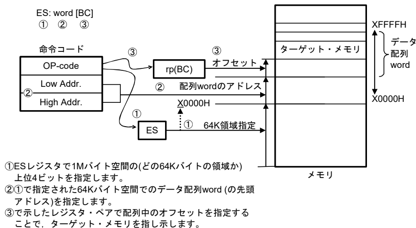
図3 - 33 ES:word[BC]の例
