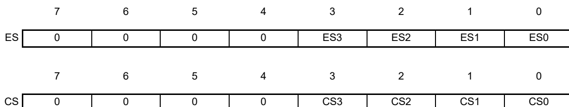
図3 - 12 ES/CS レジスタの構成
