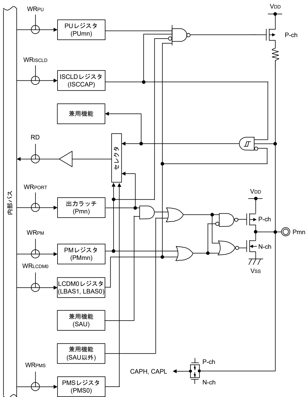
図2-10 端子タイプ7-5-5の端子ブロック図
