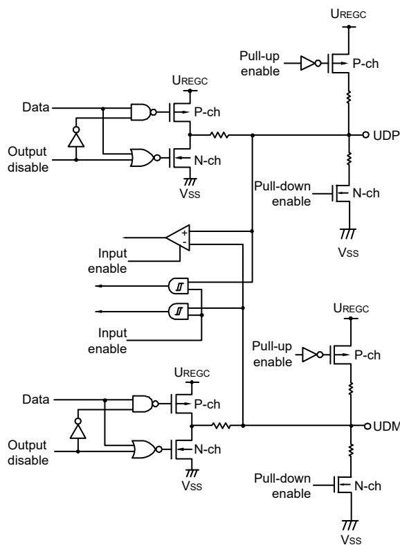
図2 - 19 端子タイプ18-11-1の端子ブロック図
