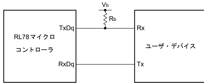
UARTモード接続図(異電位通信時)
