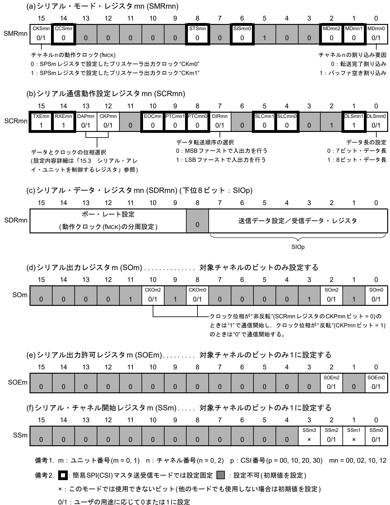
図 15 - 44 簡易SPI (CSI00, CSI10, CSI20, CSI30)のマスタ送受信時のレジスタ設定内容例
