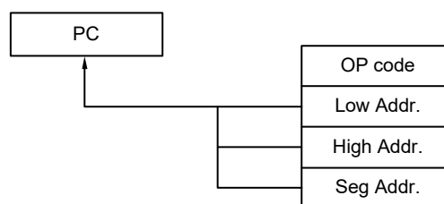
図3-15 CALL !!addr20/BR !!addr20の例
