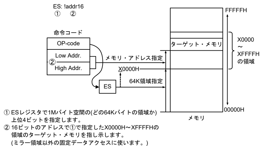
図3 - 22 ES:!addr16の例
