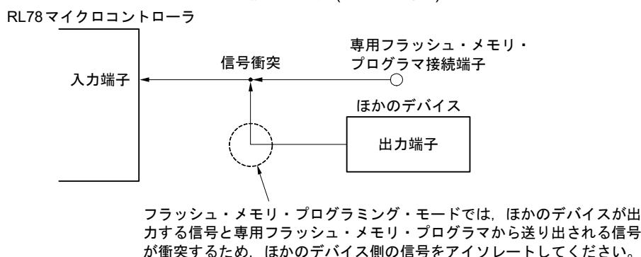
図31-5 信号の衝突(RESET端子)
