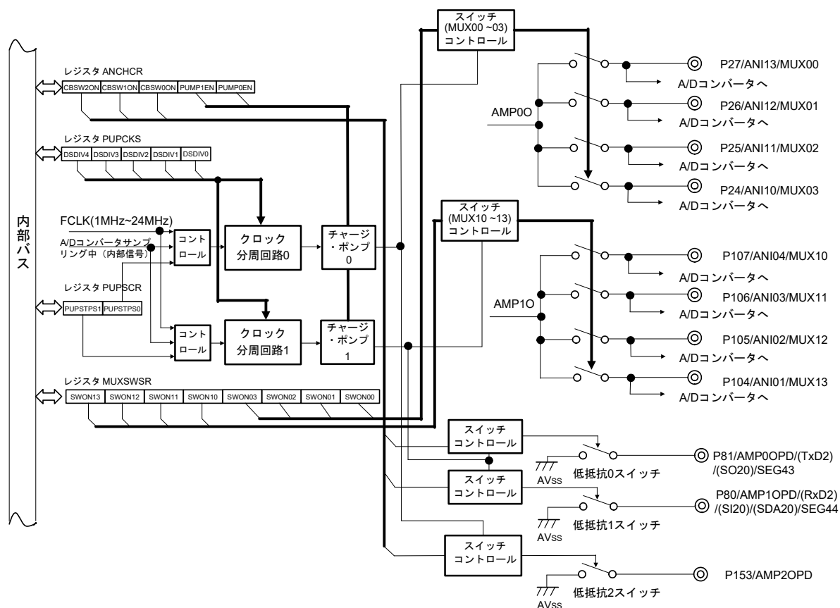
図14-2 アナログMUX & 低抵抗スイッチブロック図
