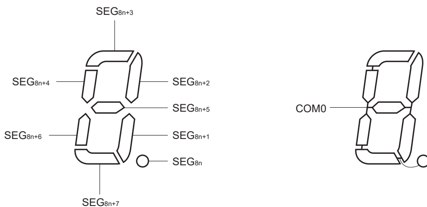
図 19 - 31 スタティックLCDの表示パターンと電極結線
