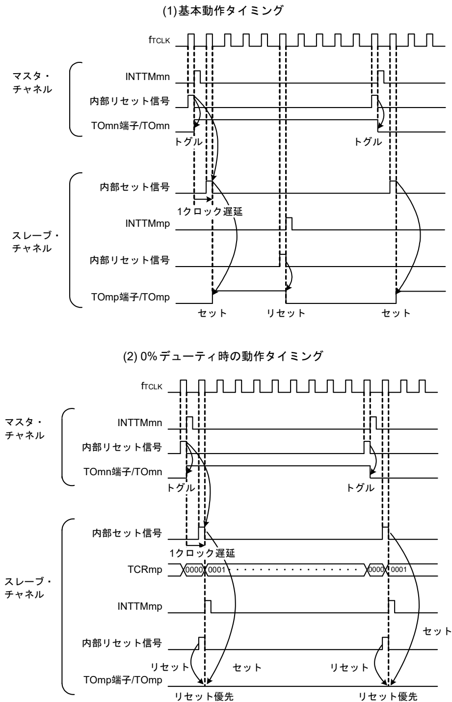
図6-41 セット/リセット・タイミング動作状態
