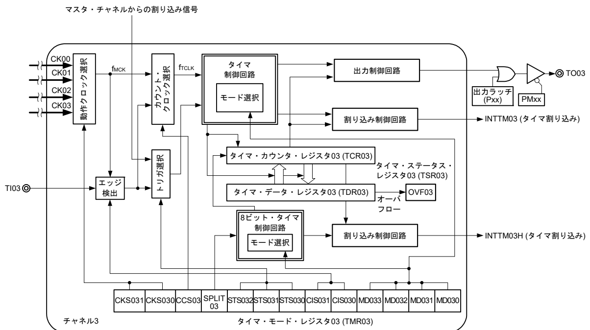
図6-5 タイマ・アレイ・ユニットのチャネル3内部ブロック図
