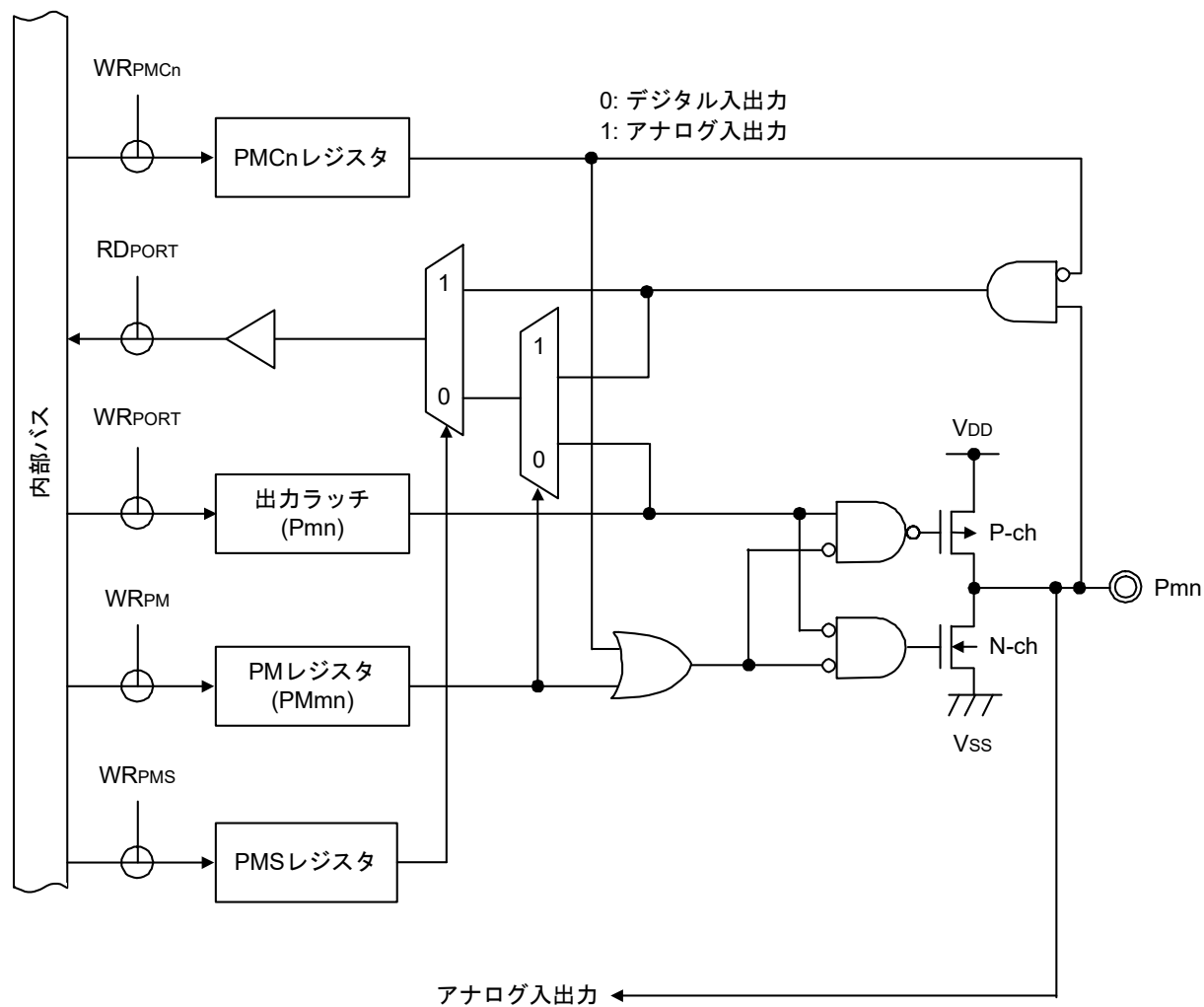
図2 - 6 端子タイプ4-3-6の端子ブロック図
