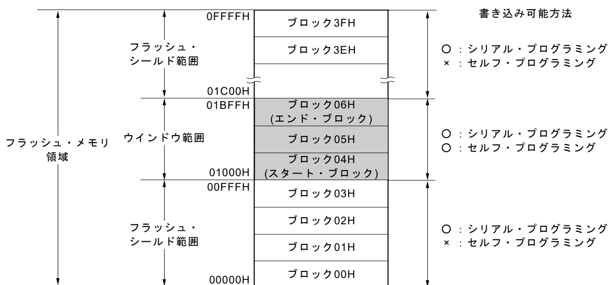
図31-11 フラッシュ・シールド・ウインドウの設定例 (対象デバイス：R5F11MME, スタート・ブロック：04H, エンド・ブロック：06Hの場合)
