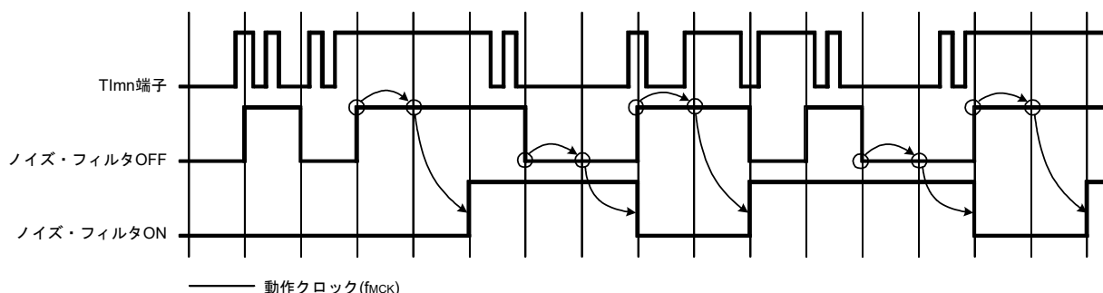
図6 - 46 Tlmn入力端子に対するノイズ・フィルタ ON/OFFによるサンプリング波形
