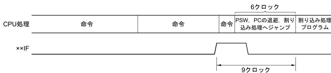
図22 - 11 割り込み要求の受け付けタイミング(最小時間)
