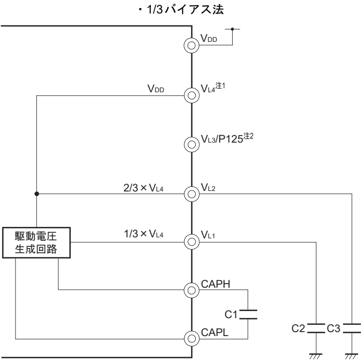
図 19 - 24 LCD駆動用電源の接続例（容量分割方式）
