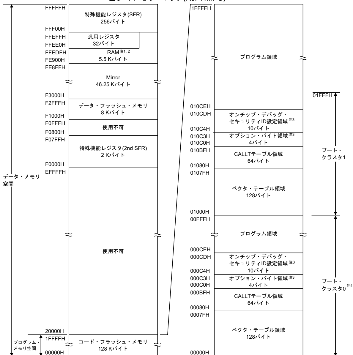
図3-4 メモリ・マップ(R5F11MPG)
