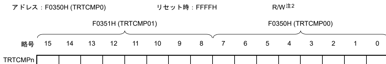
図7-5 8ビット・インターバル・タイマ・コンペア・レジスタ n (TRTCMP n )のフォーマット
