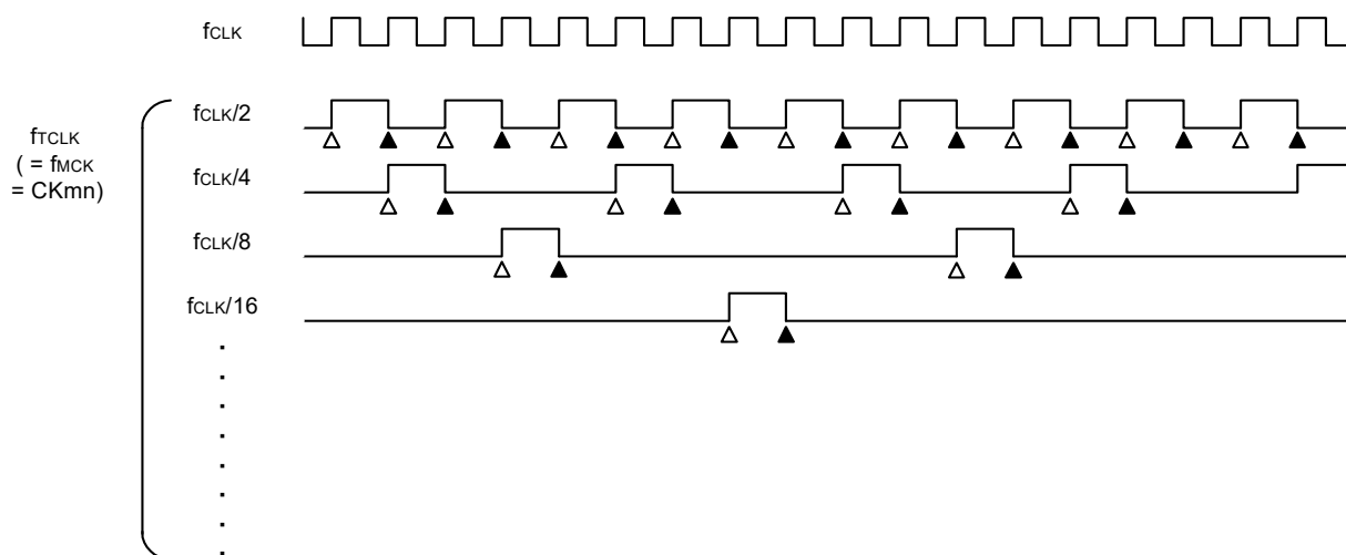
図6 - 29 f CLK とカウント・クロック (f CLK ) のタイミング (CCSmn = 0 時)
