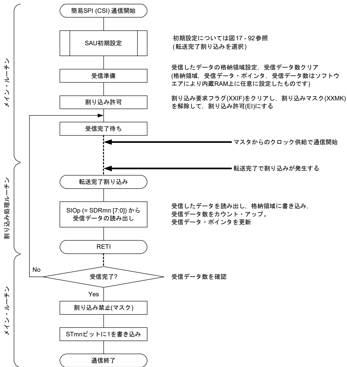
図 17 - 96 スレープ受信(シングル受信モード時)のフロー・チャート
