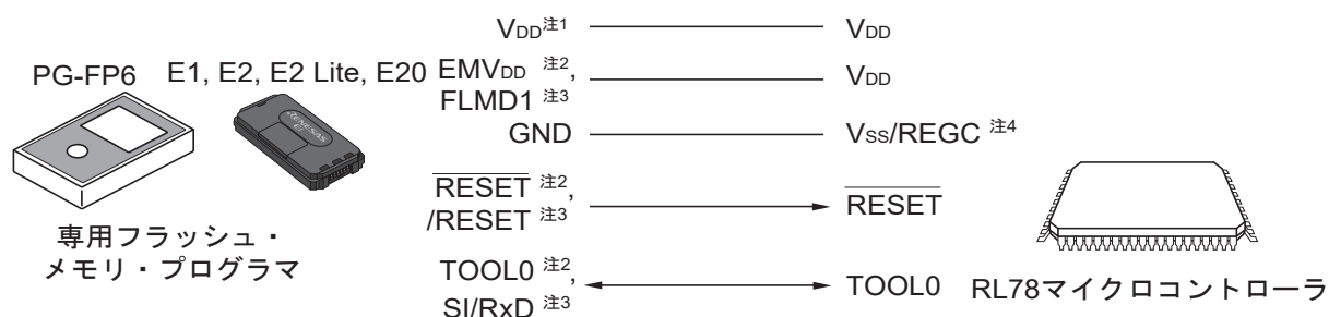
図31-2 専用フラッシュ・メモリ・プログラマとの通信
