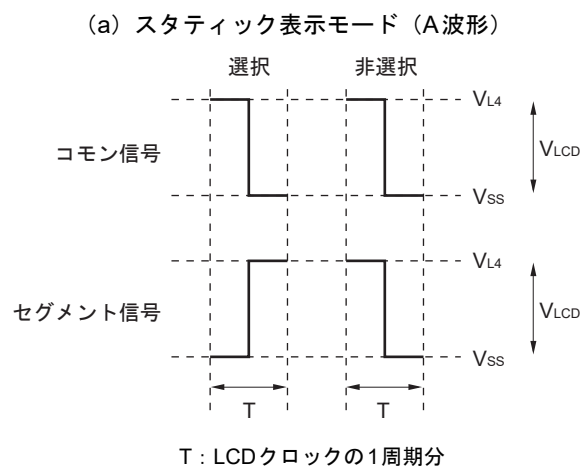
図 19 - 28 コモン信号とセグメント信号の電圧と位相 (1/3)
