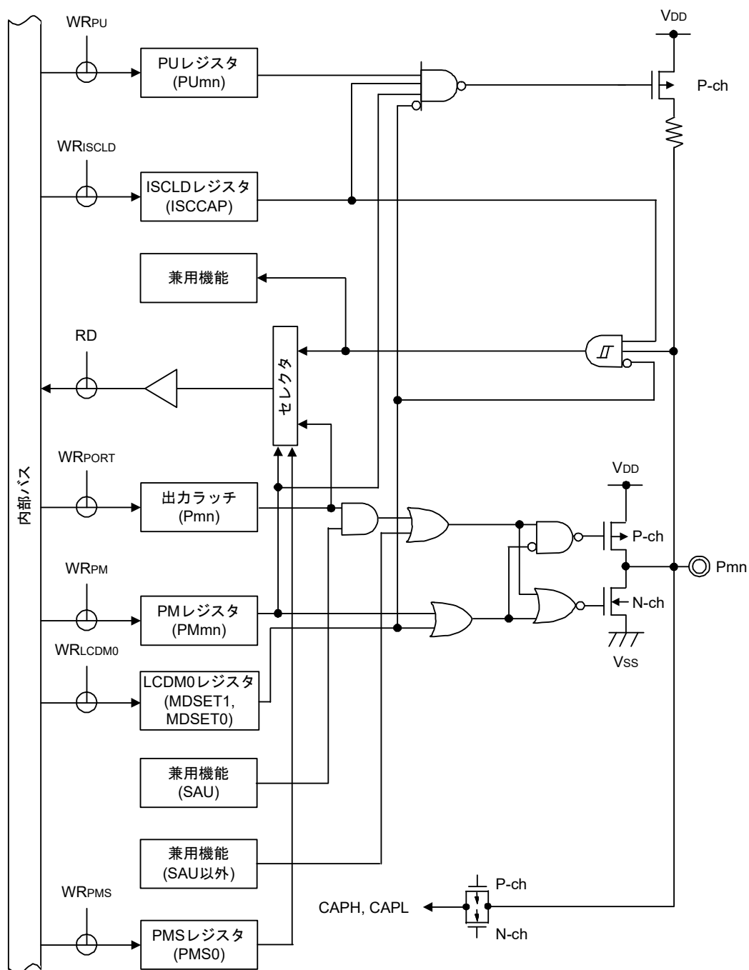
図2 - 11 端子タイプ7-5-5の端子ブロック図
