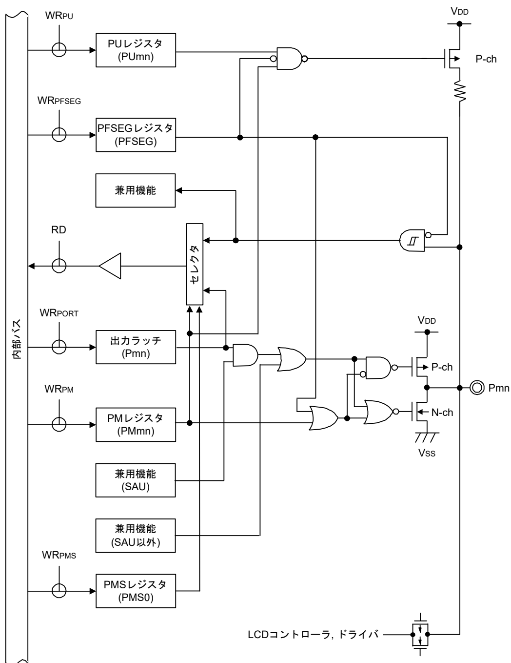
図2-10 端子タイプ7-5-4の端子ブロック図
