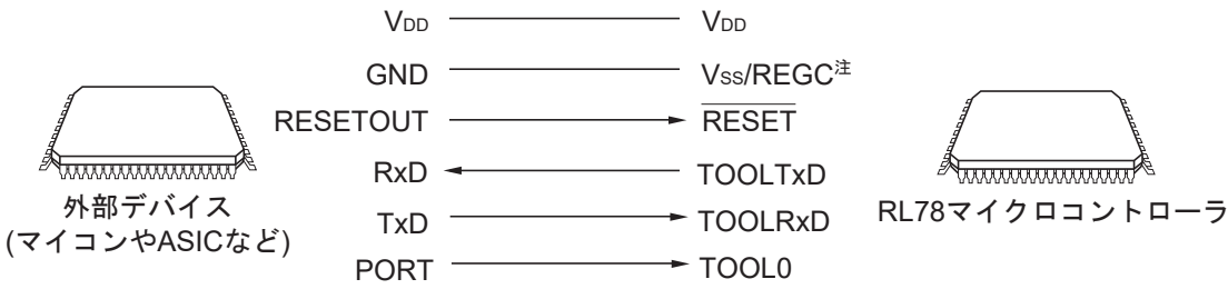
図31 - 4 外部デバイスとの通信
