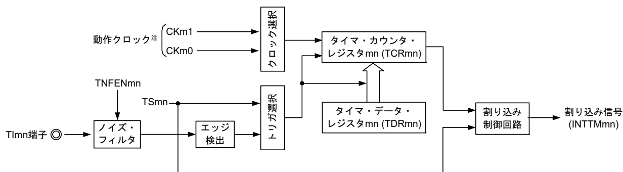
図6-64 ディレイ・カウンタとしての動作のブロック図
