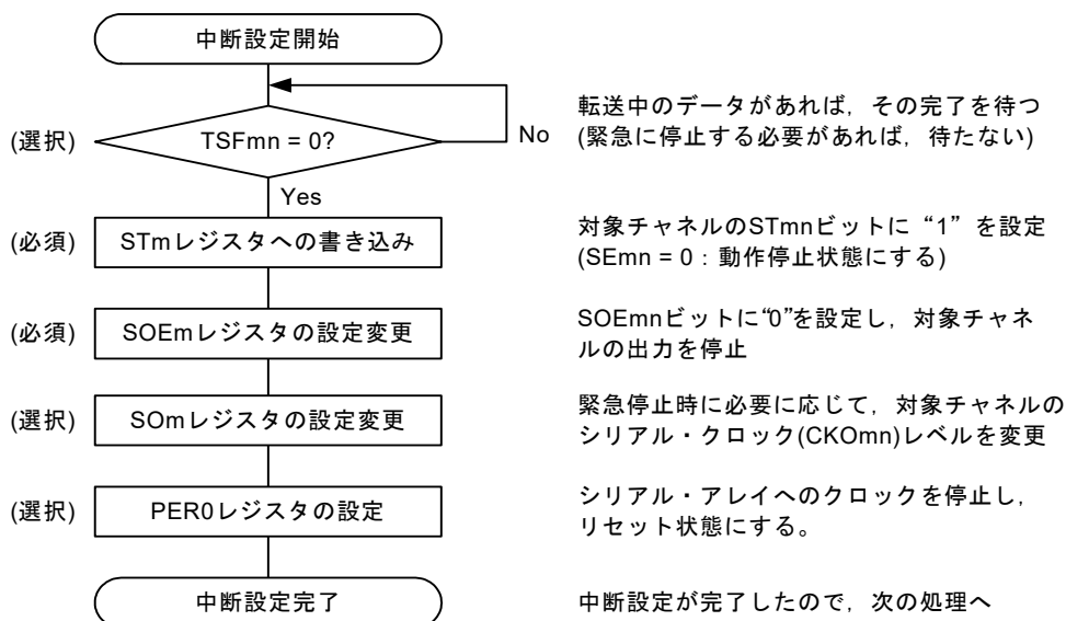
図 17 - 38 マスタ受信の中断手順
