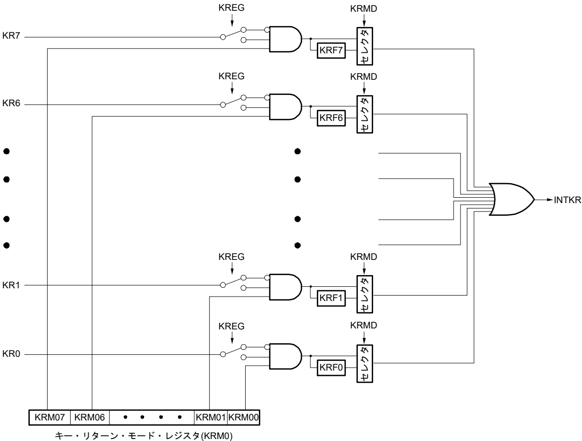
図 23 - 1 キー割り込みのブロック図
