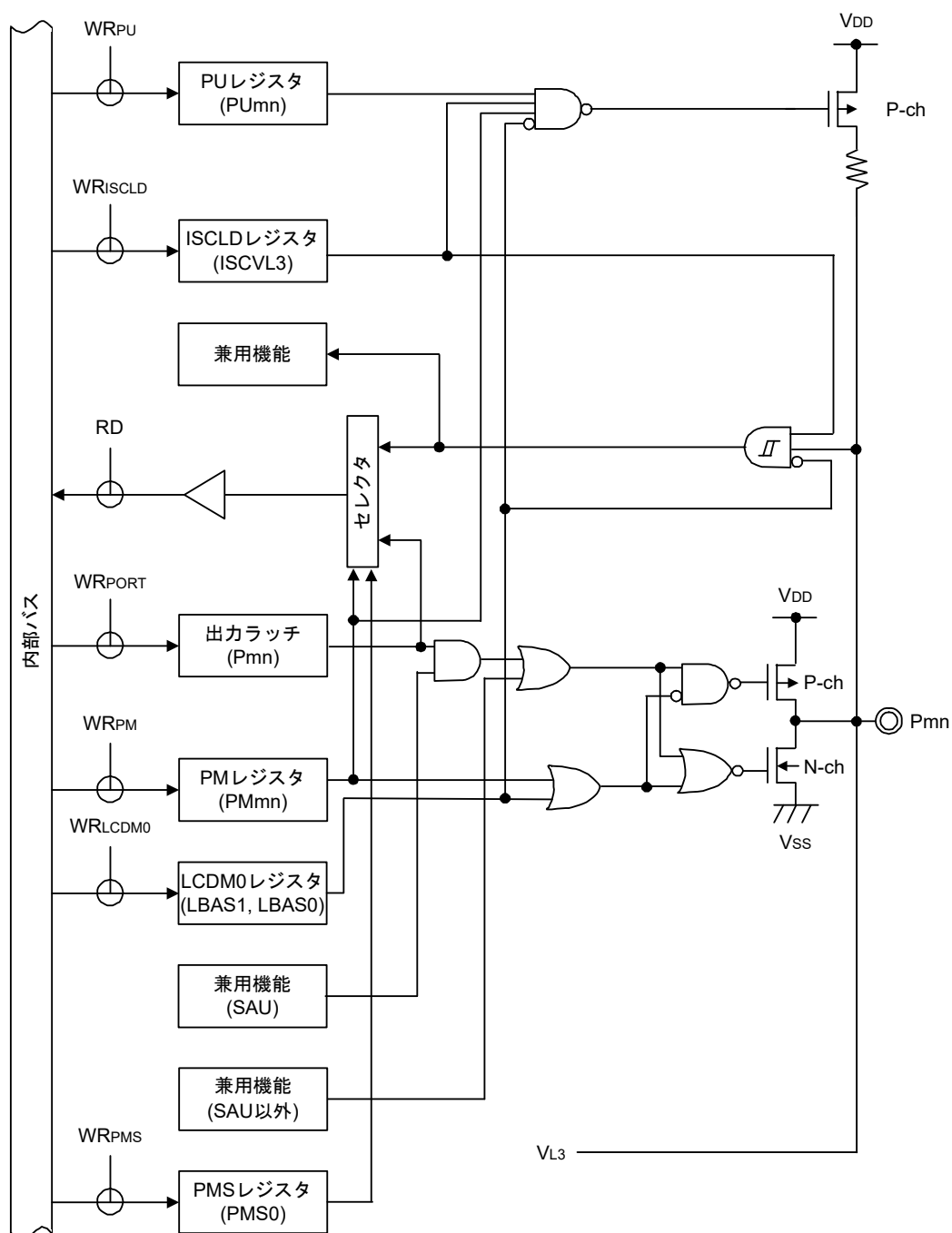
図2-12 端子タイプ7-5-6の端子ブロック図
