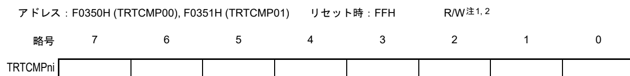
図7-4 8ビット・インターバル・タイマ・コンペア・レジスタ ni (TRTCMP ni )のフォーマット
