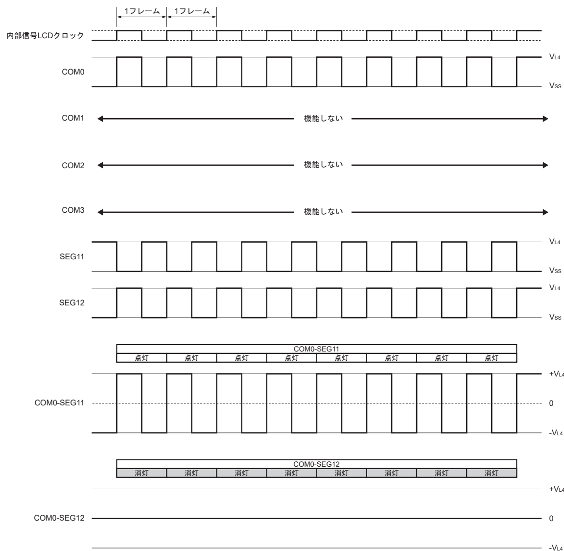
図 19 - 33 SEG11, SEG12とCOM0とのスタティックLCD駆動波形例
