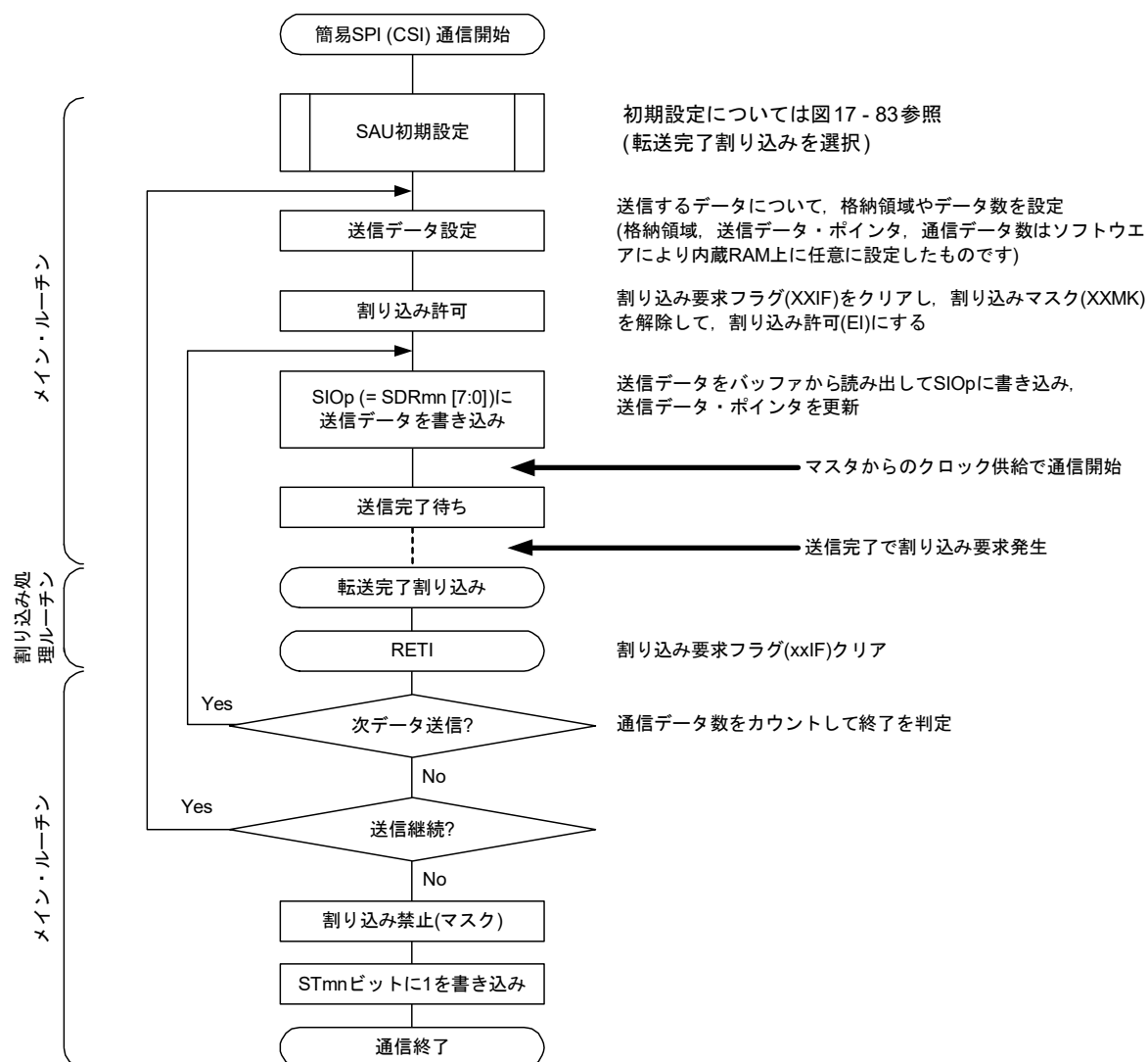
図 17 - 87 スレープ送信(シングル送信モード時)のフロー・チャート
