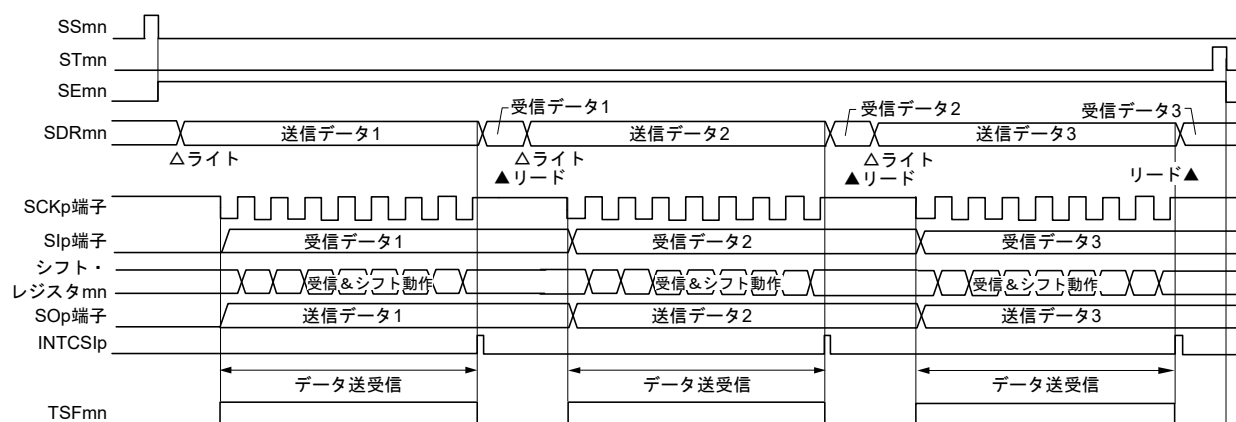
図 17 - 70 スレーブ送受信 (シングル送受信モード時) のタイミング・チャート (タイプ1 : DAPmn = 0, CKPmn = 0)
