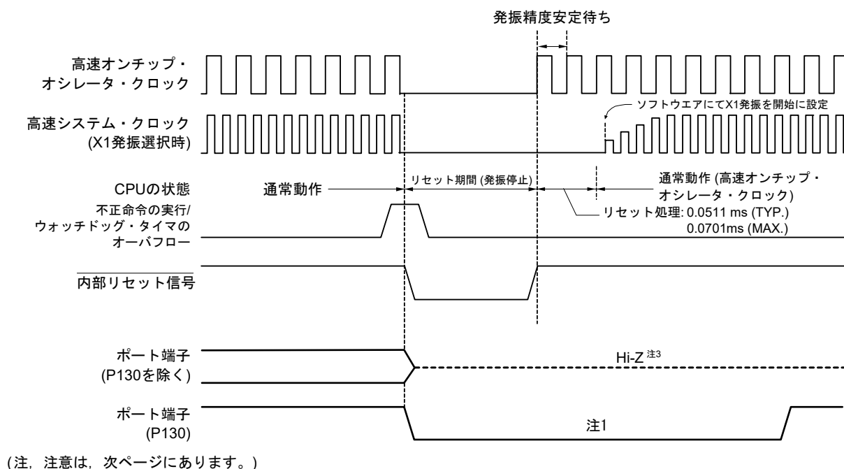
図25-3 ウォッチドッグ・タイマのオーバーフロー／不正命令の実行／RAMパリティ・エラーの検出／不正メモリ・アクセスの検出によるリセット・タイミング
