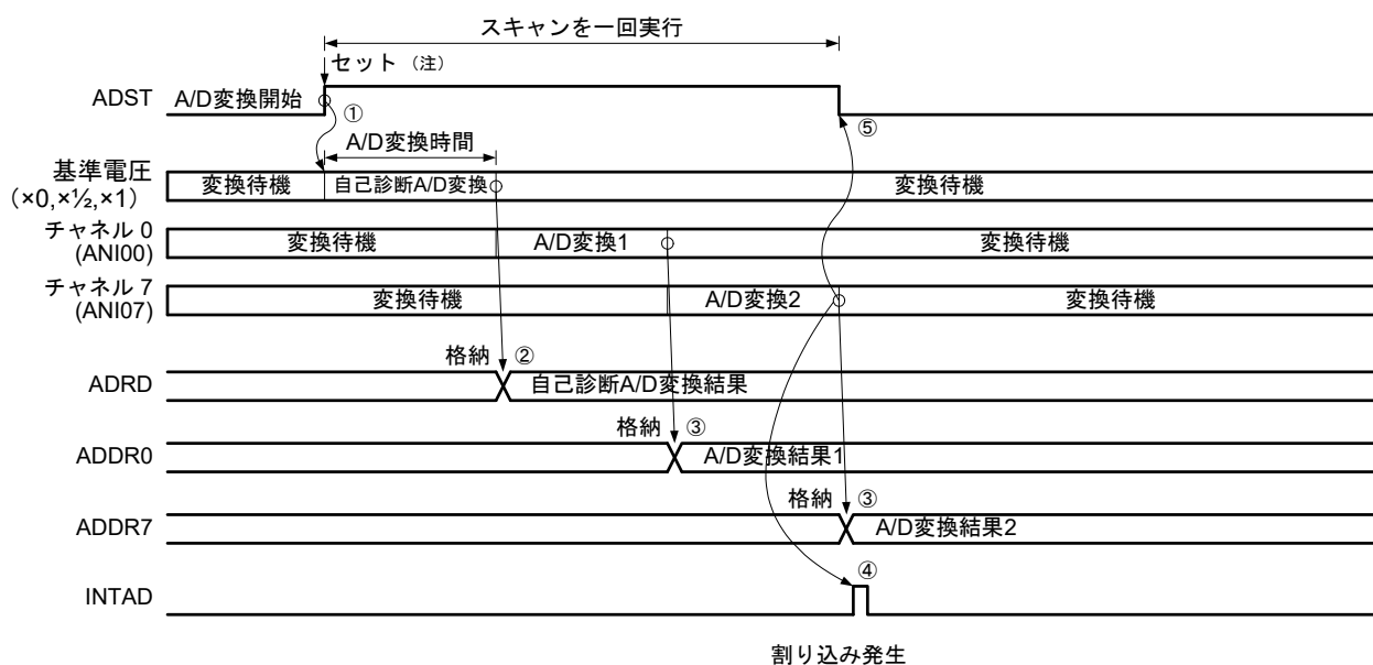
図12-18 シングルスキャンモードの動作例（基本動作：ANI00, ANI07選択 + 自己診断）
