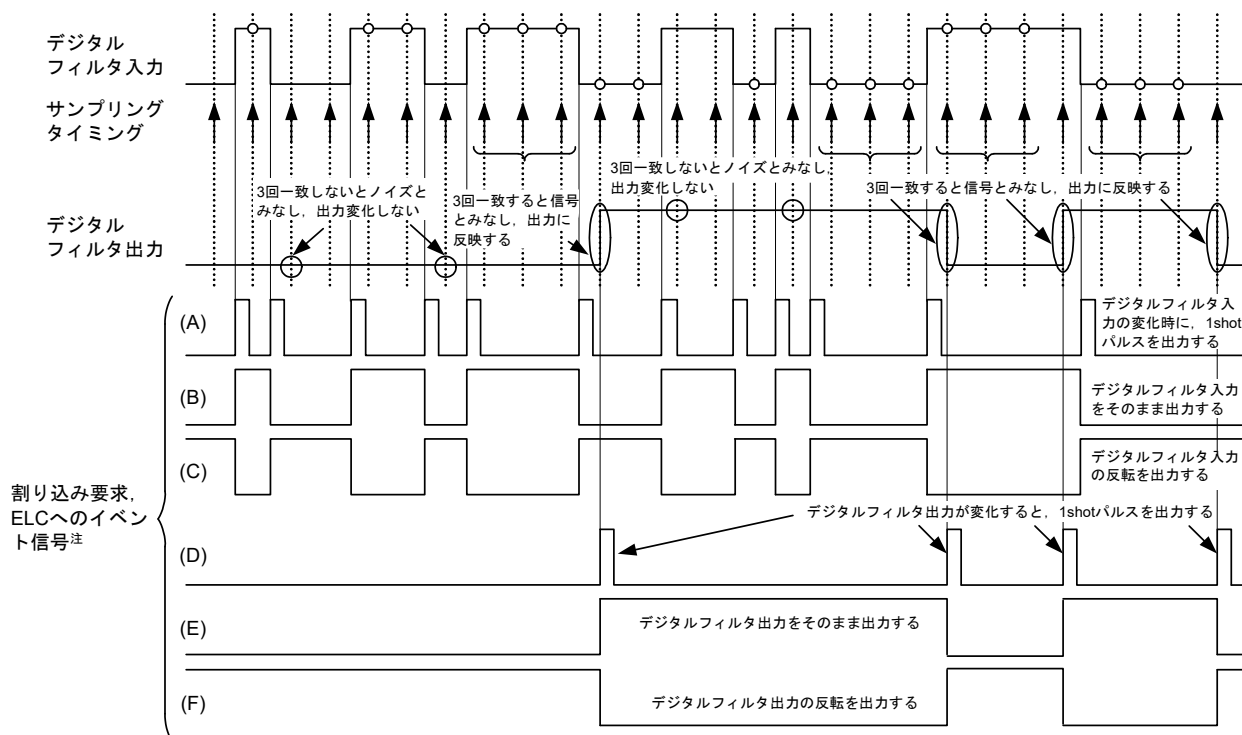
図 16 - 11 デジタルフィルタと割り込み要求・ELCへのイベント信号出力動作
