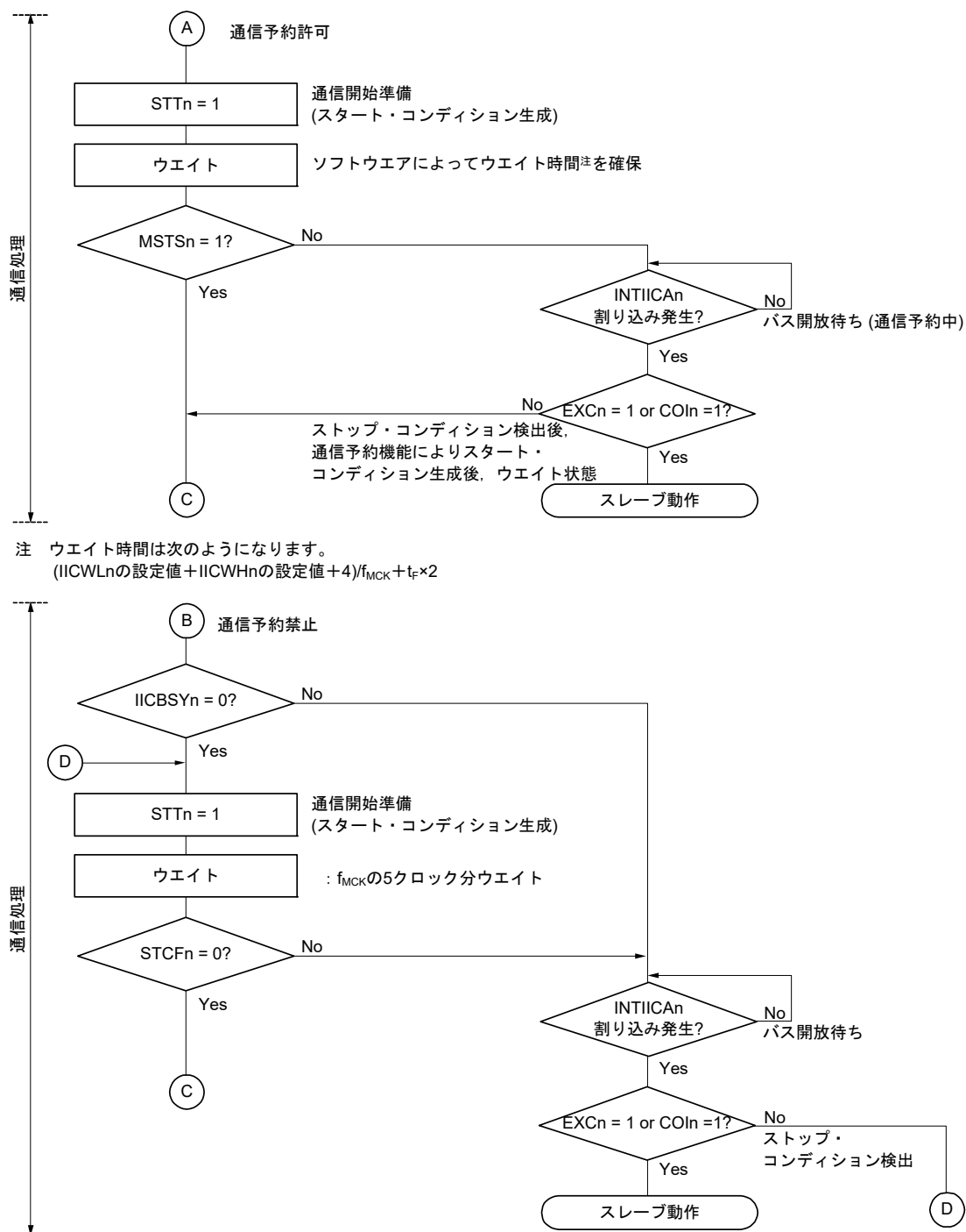
図18-37 マルチマスタ・システムでのマスタ動作(2/3)
