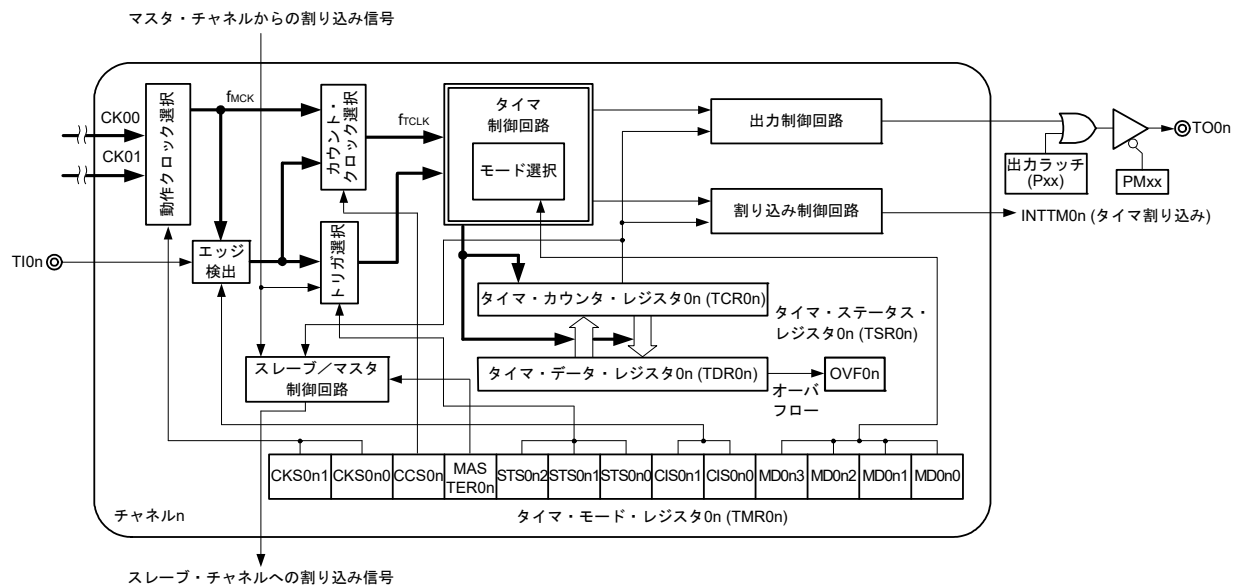
図6-4 タイマ・アレイ・ユニットのチャネルn内部ブロック図
