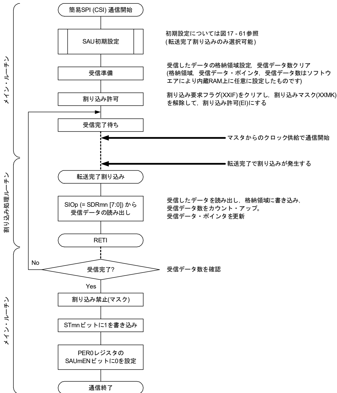
図17 - 65 スレープ受信(シングル受信モード時)のフロー・チャート
