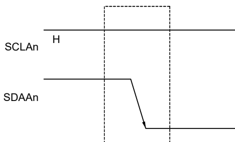
図18-21 スタート・コンディション
