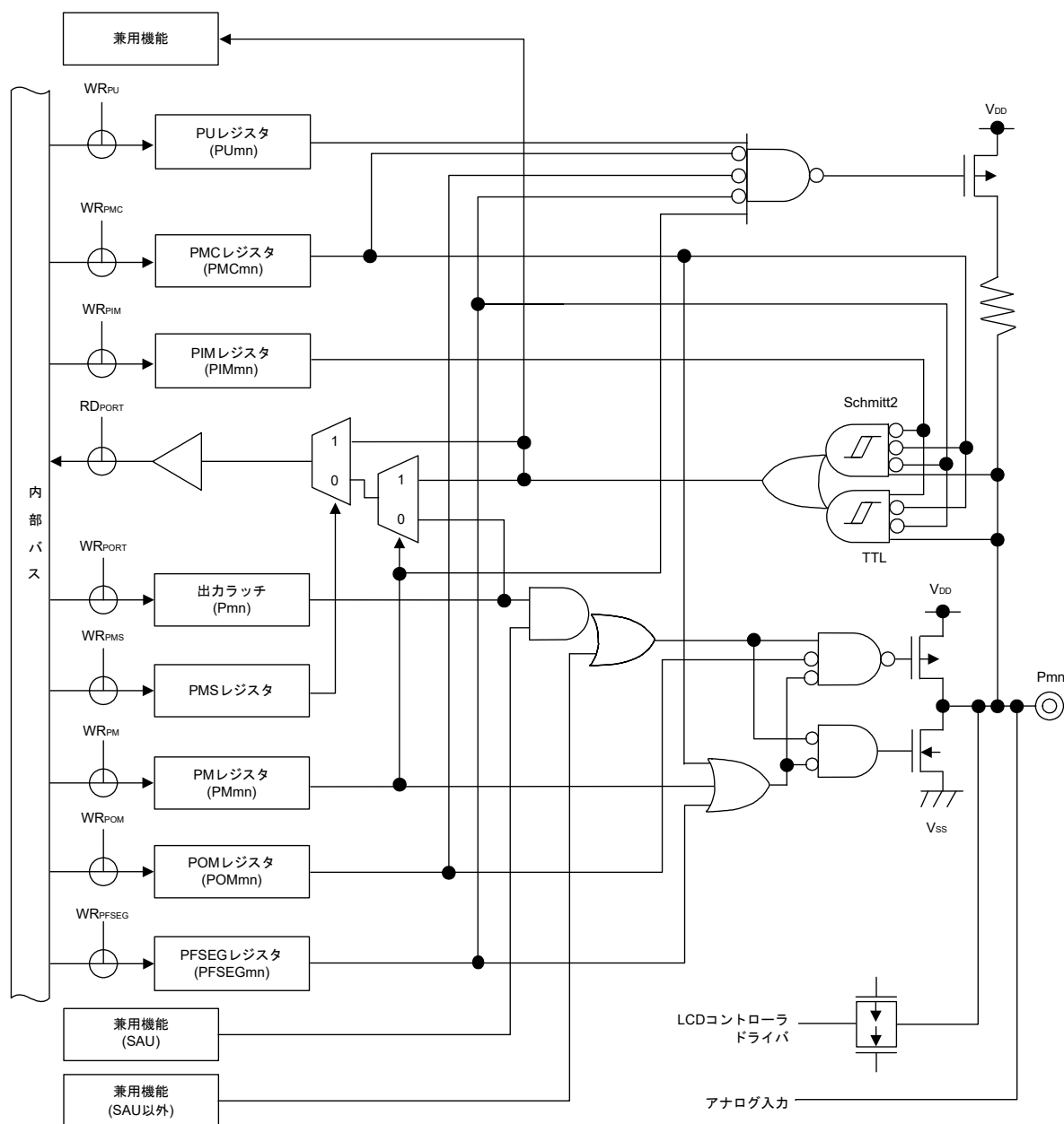
図2 - 18 端子タイプ8-5-13の端子ブロック図
