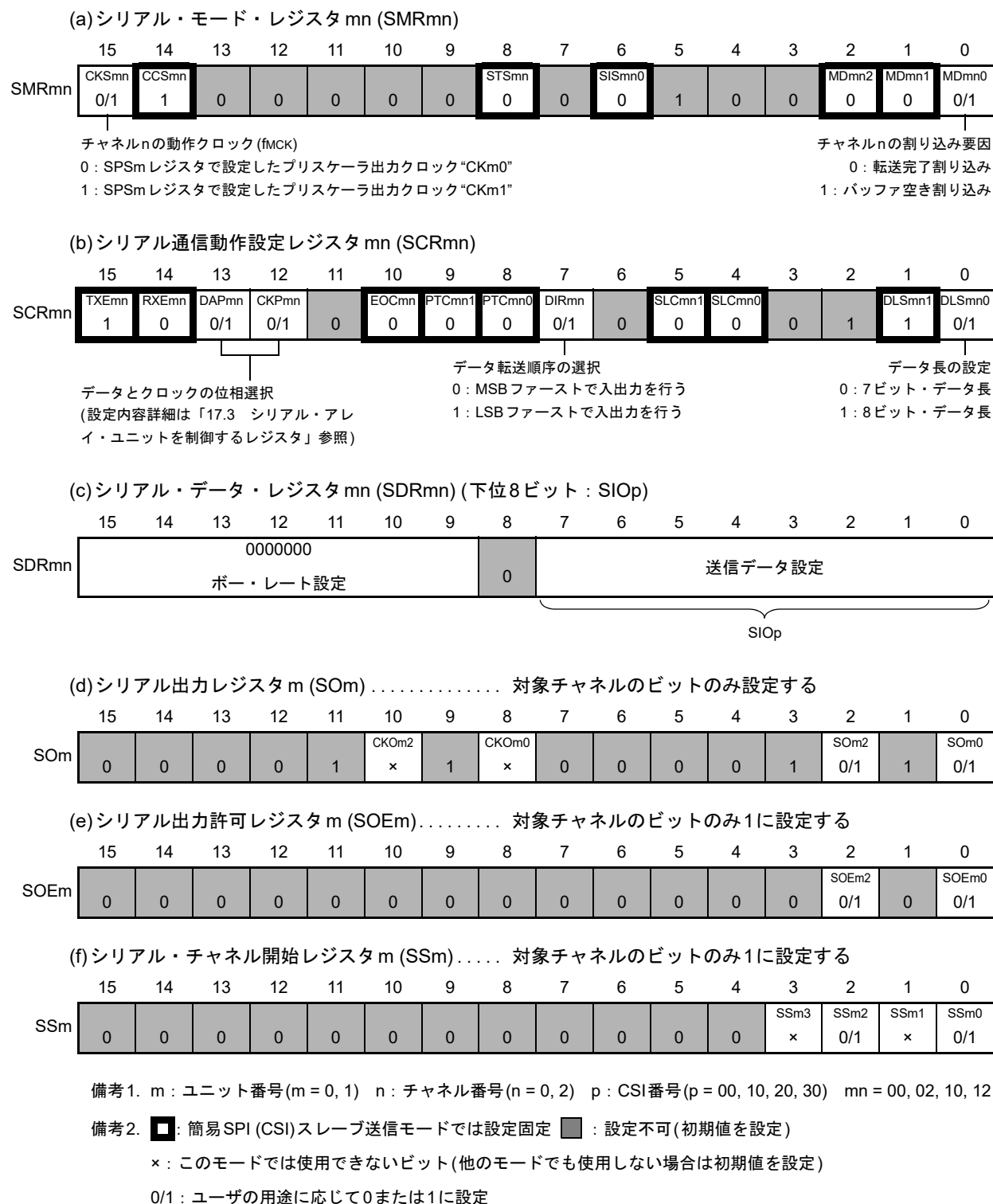
図 17 - 52 簡易 SPI (CSI00, CSI10, CSI20, CSI30)のスレーブ送信時のレジスタ設定内容例
