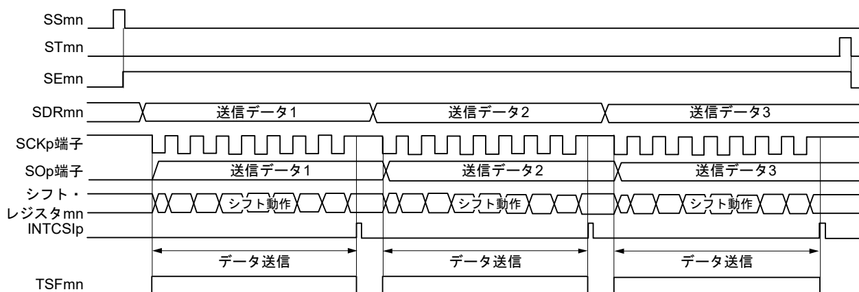
図 17 - 32 マスタ送信 (シングル送信モード時)のタイミング・チャート (タイプ1 : DAPmn = 0, CKPmn = 0)
