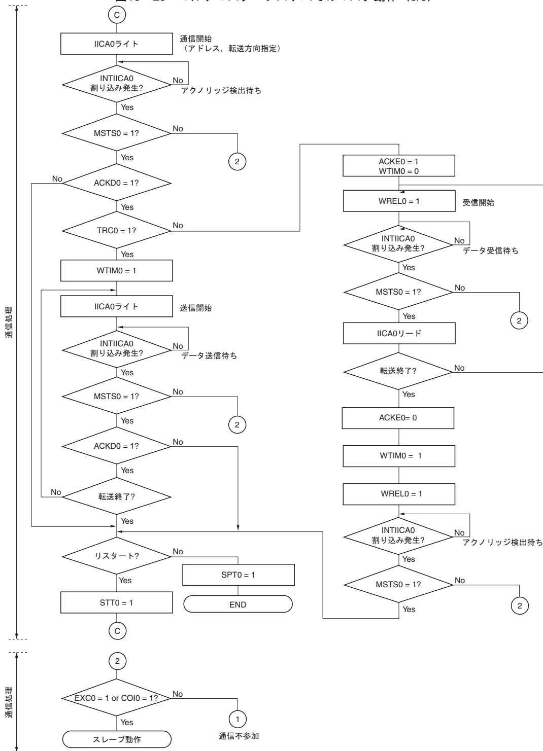
図13-29 マルチマスタ・システムでのマスタ動作 (3/3)
