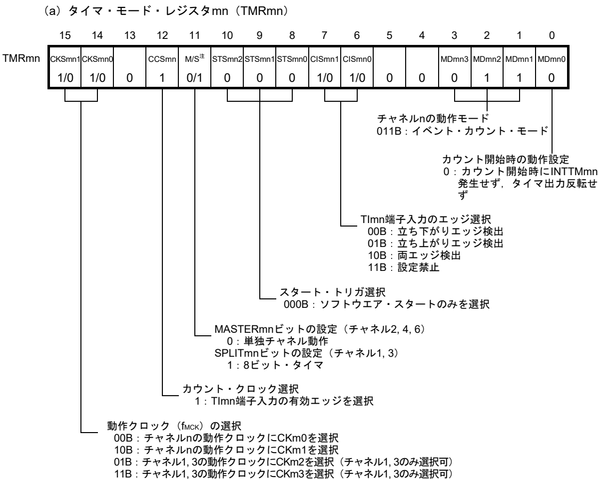
図6-51 外部イベント・カウンタ・モード時のレジスタ設定内容例
