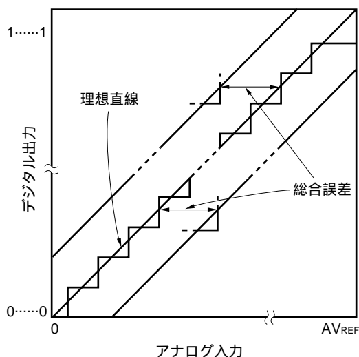
図11-33 総合誤差
