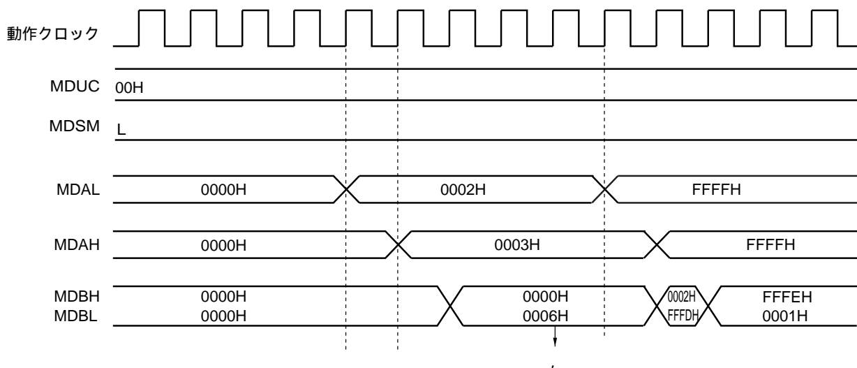
図15-6 乗算（符号なし）動作のタイミング図（ 2 \times 3 = 6 ）
