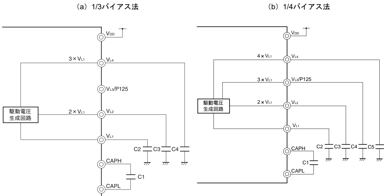
図14-23 LCD駆動用電源の接続例（内部昇圧方式）
