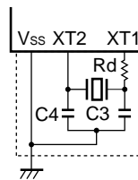
(b) XT1発振
