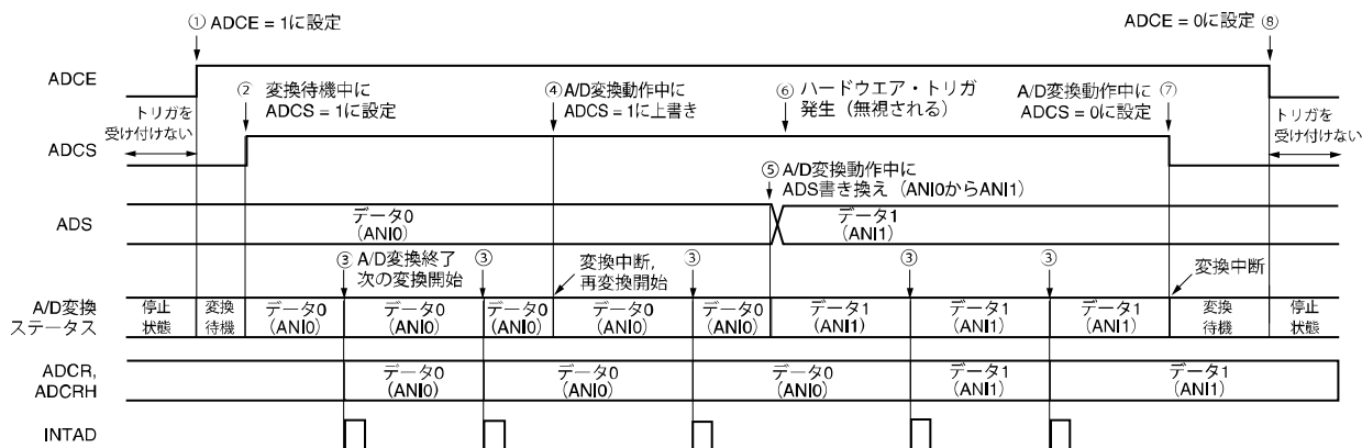
図11-17 ソフトウェア・トリガ・モード（連続変換モード）動作タイミング例
