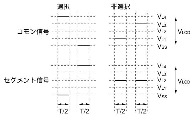
(f) 1/4バイアス法 (B波形)
