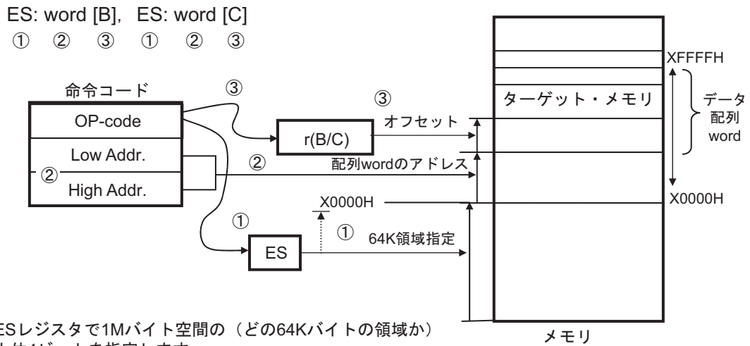
図3-31 ES:word[BC]の例
