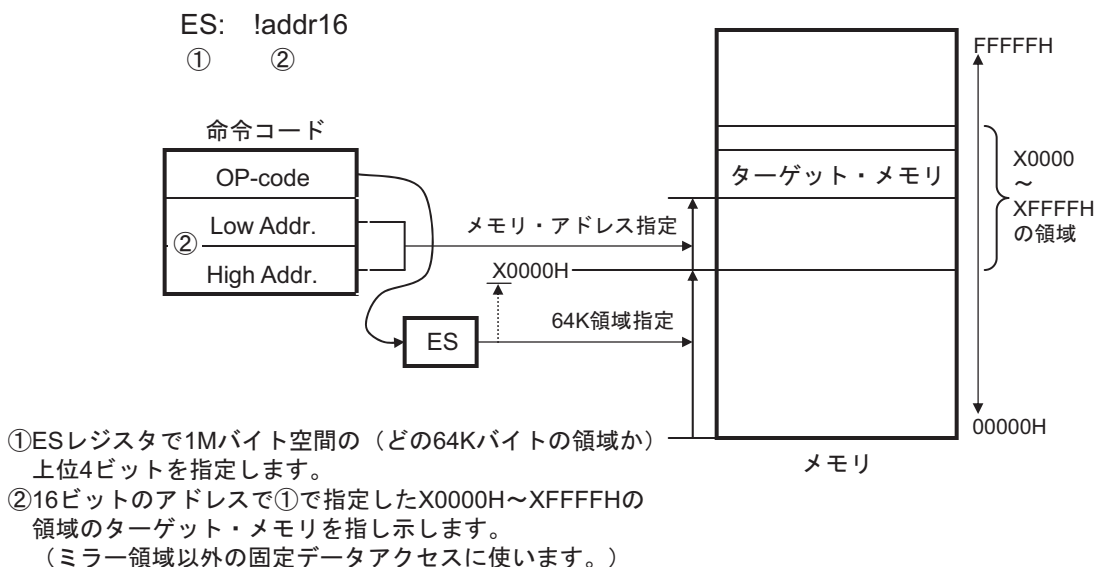
図3-20 ES:ADDR16の例
