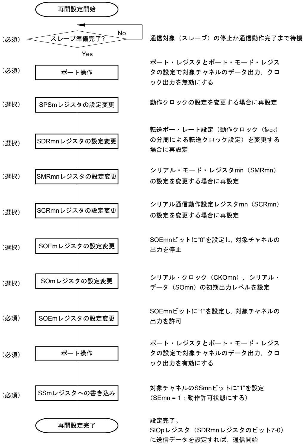
図12-26 マスタ送信の再開設定手順
