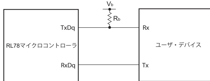
UARTモード接続図 (異電位通信時)
