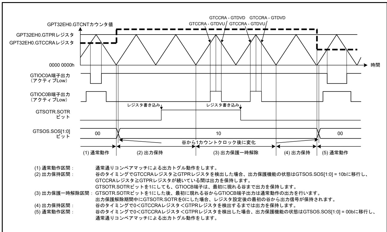
図 23.106 谷でのバッファ転送中に GTCCR レジスタ \geq GTPR レジスタとなった場合の出力保護機能一時解除例 (谷でのバッファ転送中に 0 < \text{GTCCR レジスタ} < \text{GTPR レジスタ} を回復、アクティブ Low の場合)
