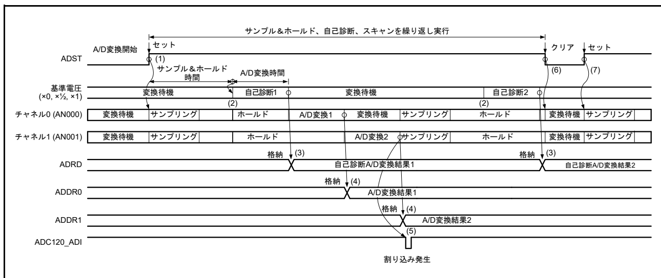
図 45.20 連続スキャンモードの動作例 (チャンネル専用サンプル&ホールド回路使用、AN000 および AN001 選択 + 自己診断)
