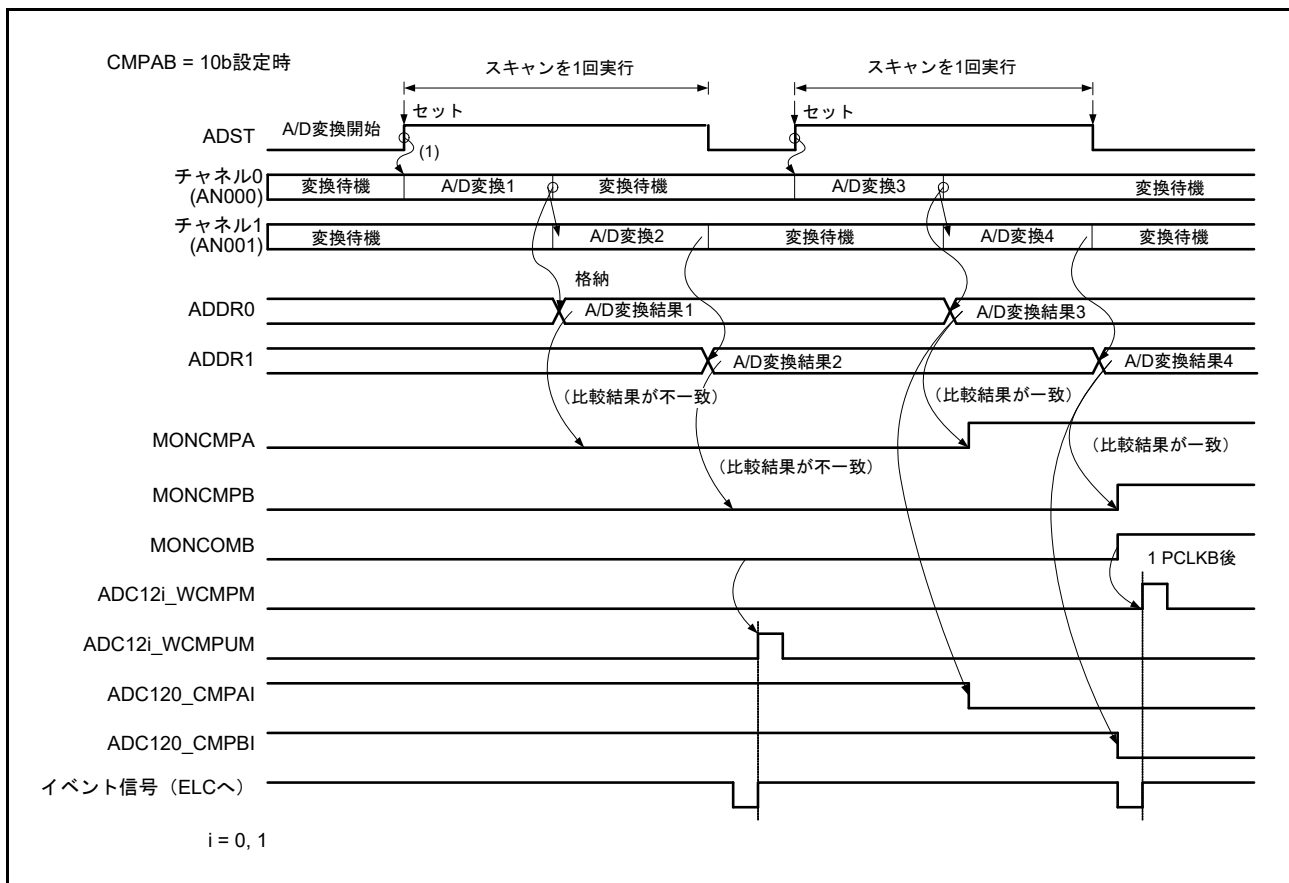
図 45.33 コンペア機能のイベント出力動作例 (AN000 ~ AN001 を比較)
