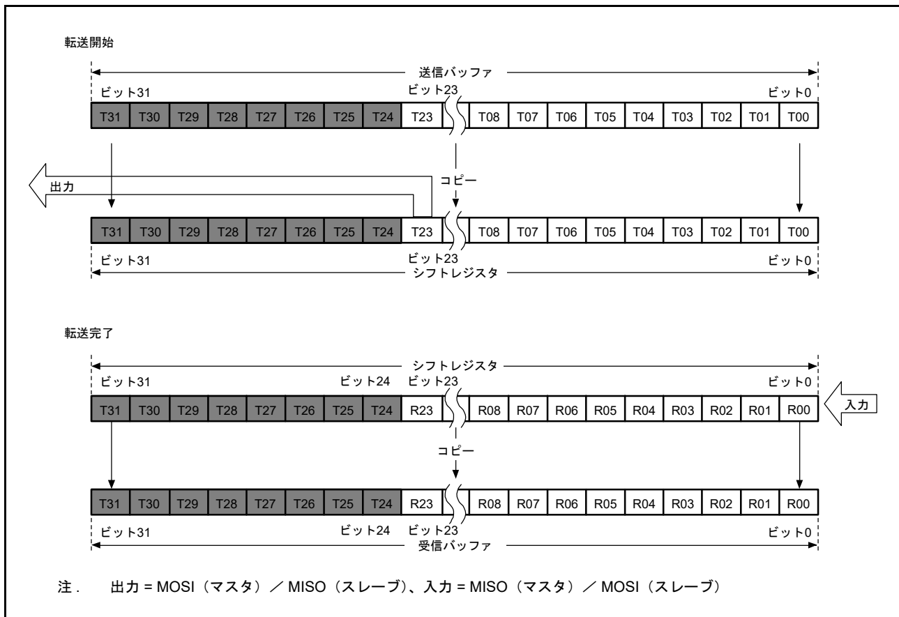
図 36.15 MSB ファースト転送 (24 ビットデータ/パリティ機能無効)
