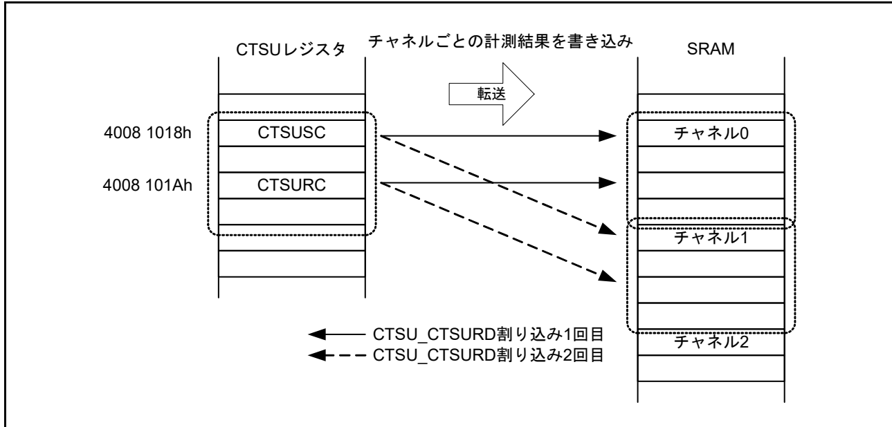
図 49.20 CTSU_CTSURD 割り込みを用いた DTC 転送動作例
