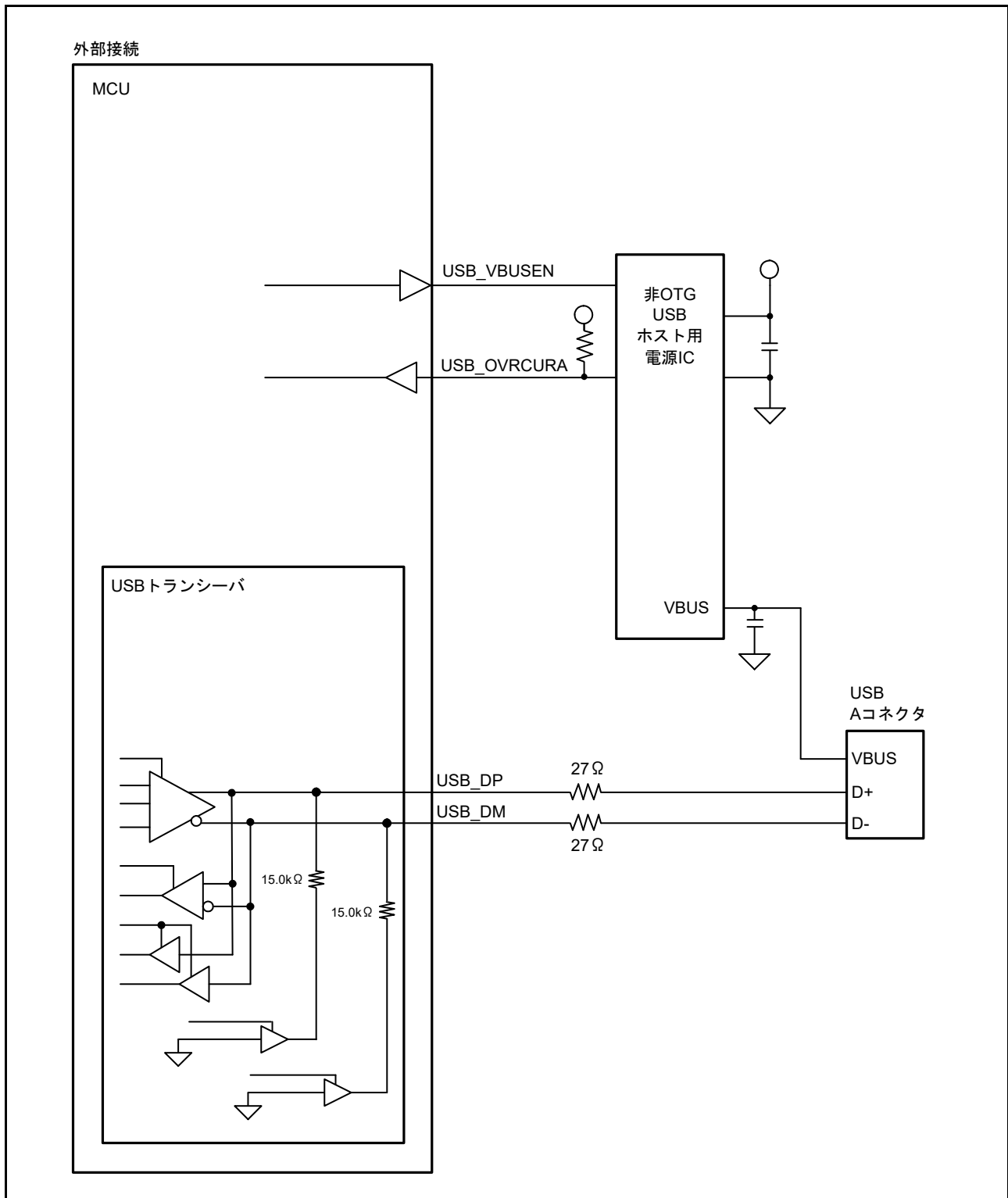
図 31.4 ホスト接続例
