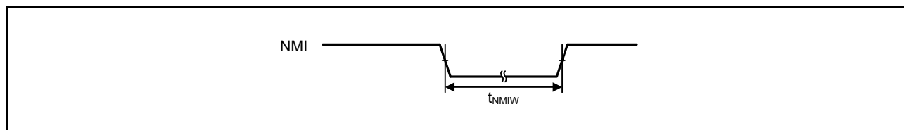
図 55.18 NMI 割り込み入カタイミング
