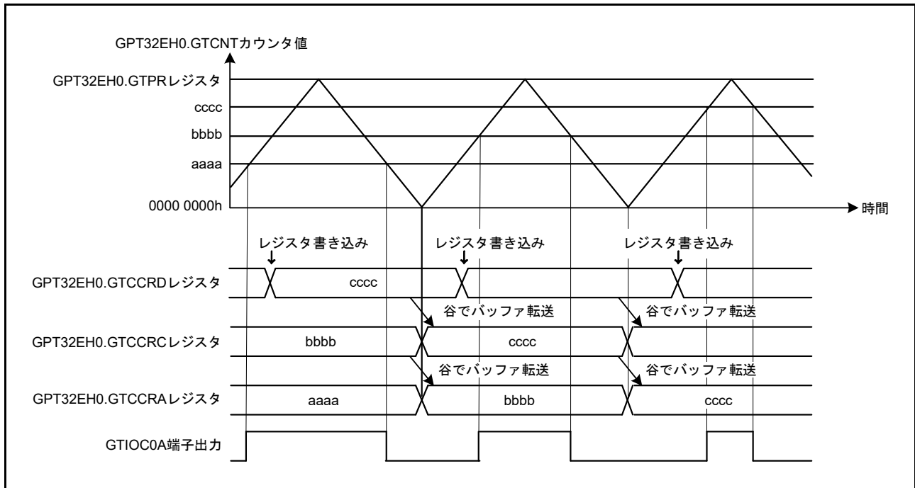
図 23.23 GTCCRA、GTCCRB レジスタのダブルバッファ動作例 (アウトプットコンペア、三角波、谷でバッファ動作、GTCCRA レジスタのコンペアマッチでトグル出力、周期の終わりで出力保持の場合)
