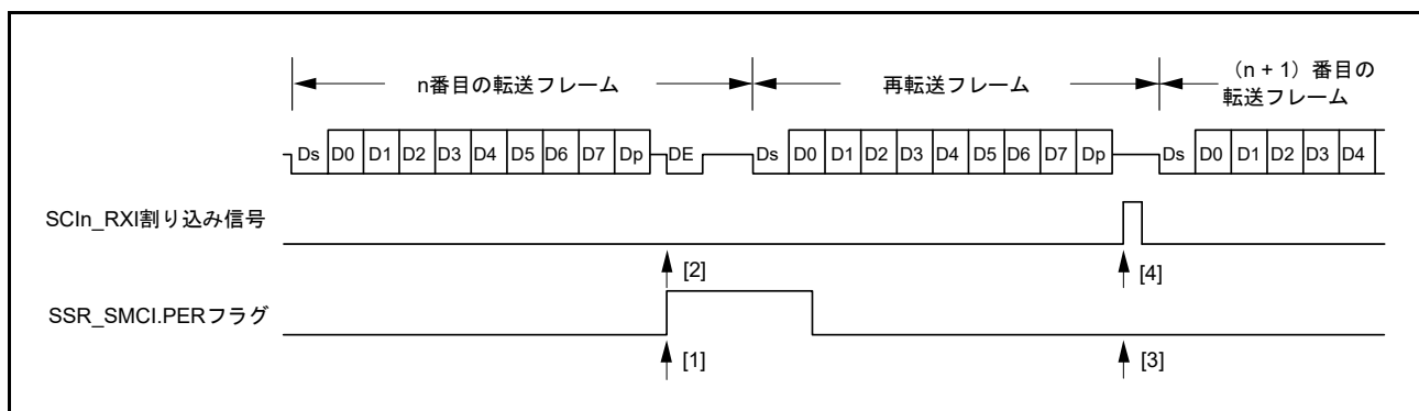
図 32.55 SCI 受信モードでの再転送動作
