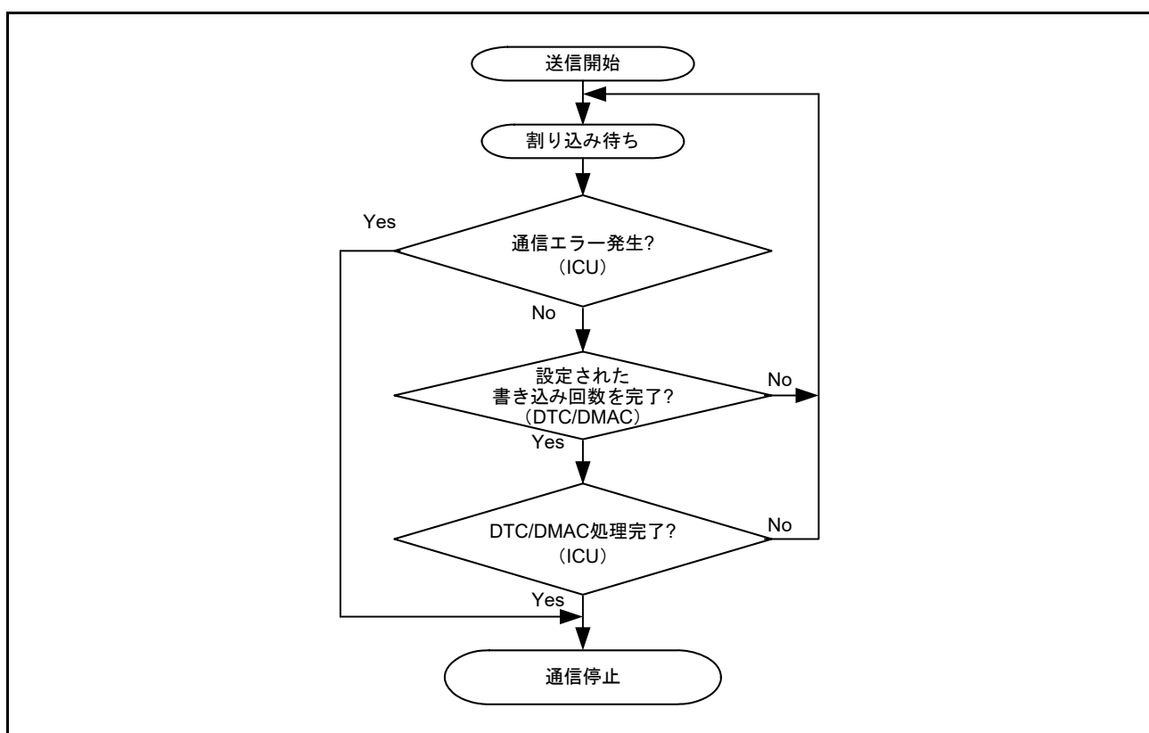
図 39.54 送信手順
