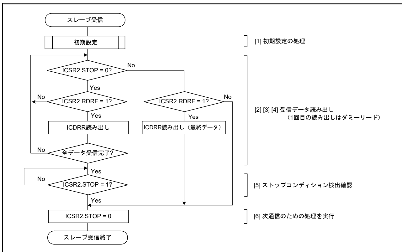
図 34.18 スレーブ受信のフロー例
