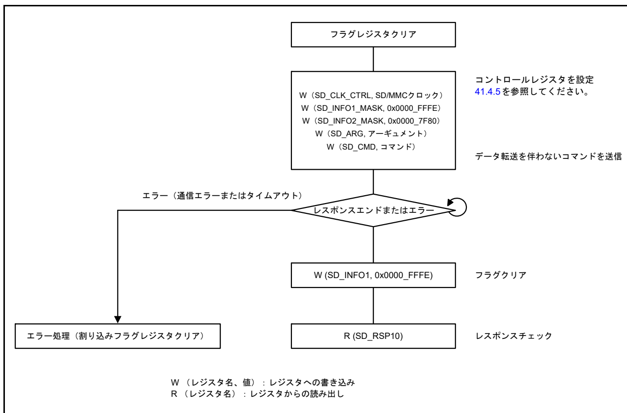
図 41.10 データがないコマンドのフロー例
