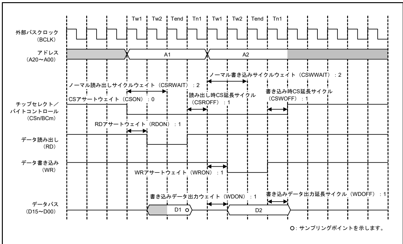
図 15.13 ノーマルアクセスの動作例（読み出し／書き込み）（ n = 0 \sim 7 および m = 0, 1 ）
