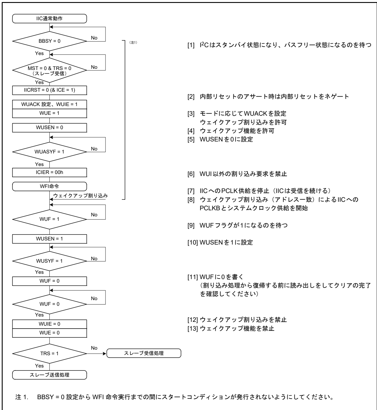
図 34.30 ノーマルウェイクアップモード1の動作例 (スレープアドレス一致時のウェイクアップ割り込みによるウェイクアップの場合)
