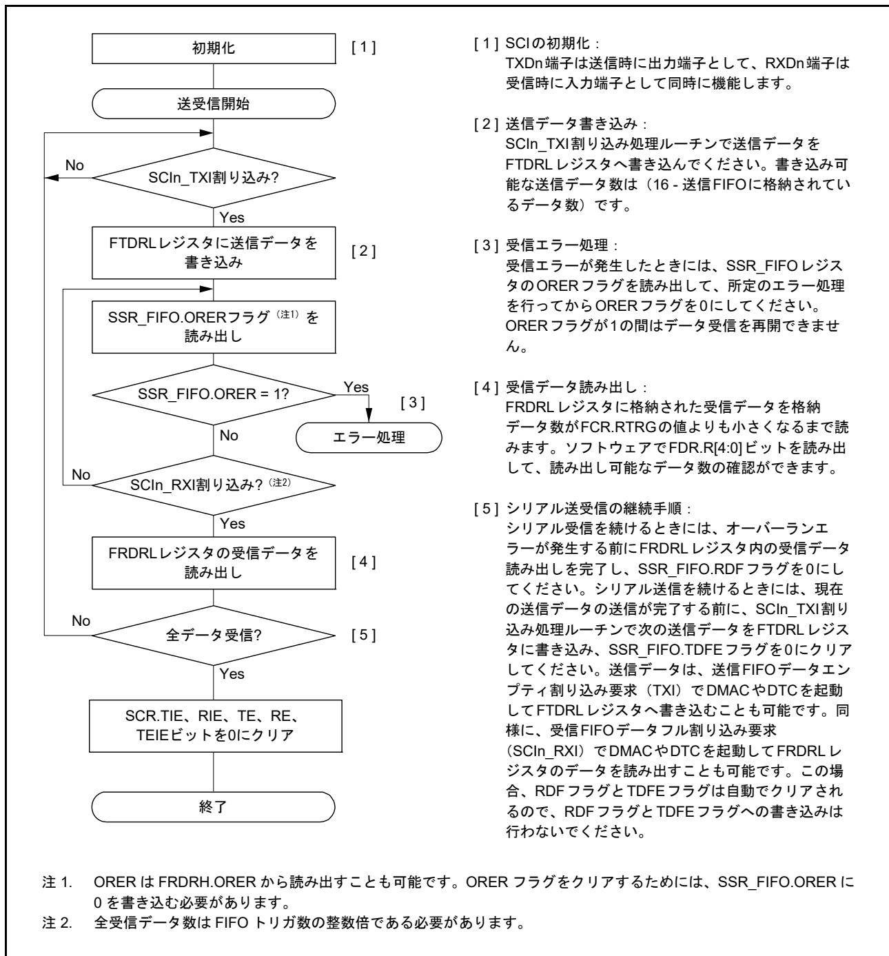
図 32.44 クロック同期モードにおけるシリアル同時送受信動作のフローチャート例 (FIFO 選択時)
