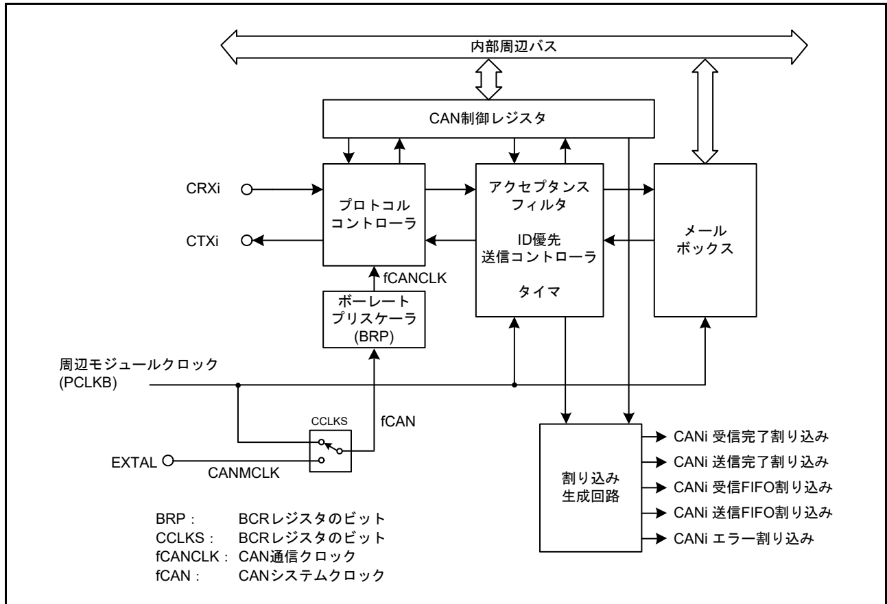
図 35.1 CANモジュールブロック図 (i = 0, 1)
