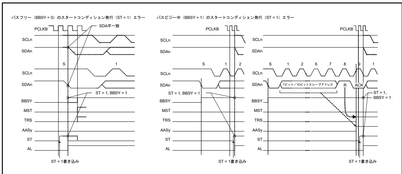
図 34.42 スタートコンディション発行時のアビトラージョンロスト (MALE = 1 の場合)
