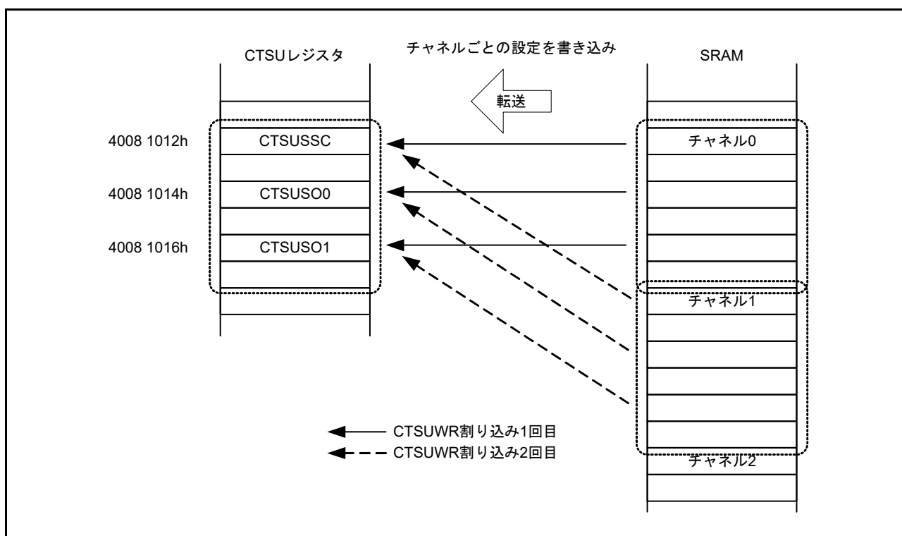
図 49.19 CTSUS_CTSUWR 割り込みを用いた DTC 転送動作例
