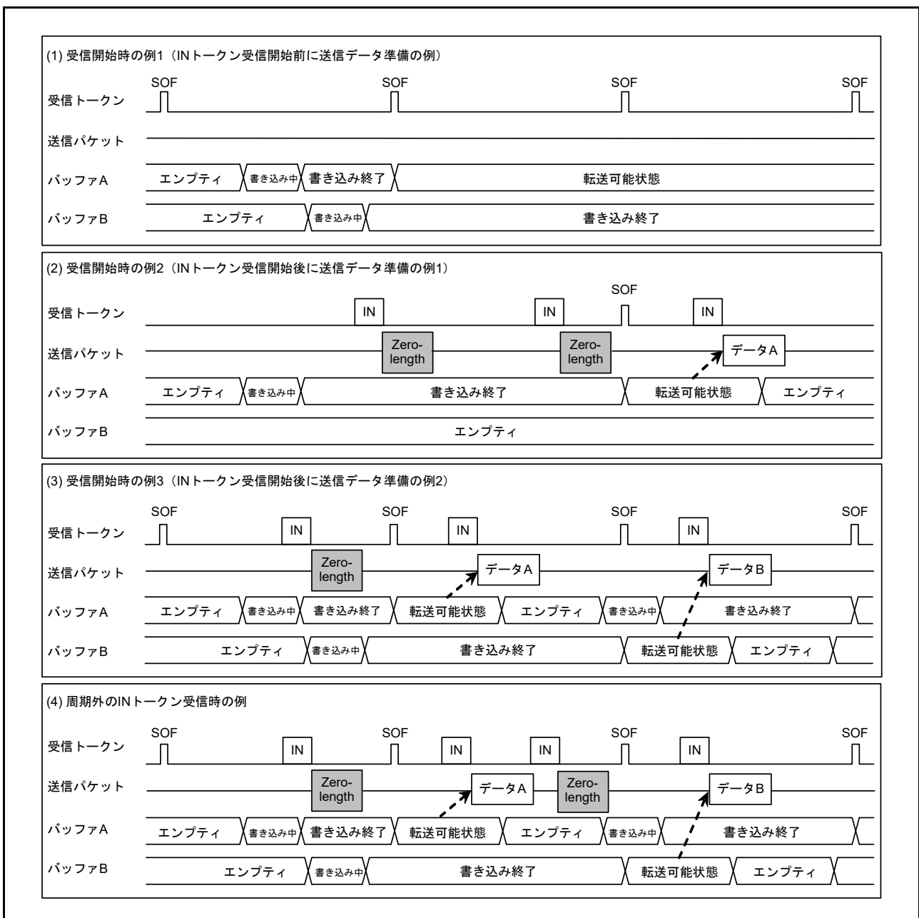
図 31.20 データセットアップ動作例
