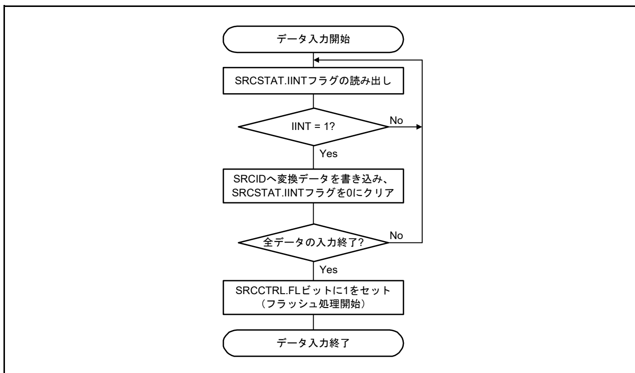
図 40.3 データ入力フロー
