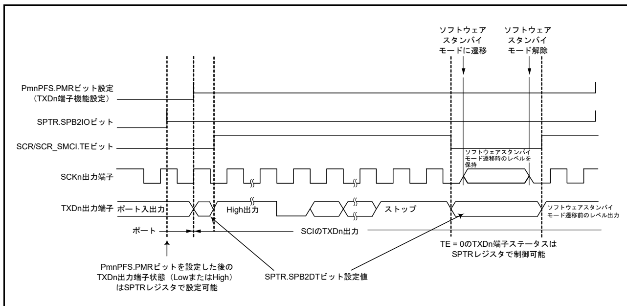
図 32.74 ソフトウェアスタンバイモード遷移中のポートの端子状態 (内部クロック、調歩同期送信)
