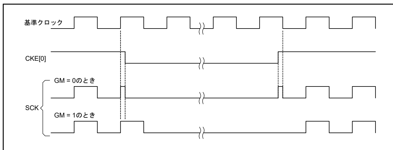
図 32.57 クロック出力制御
