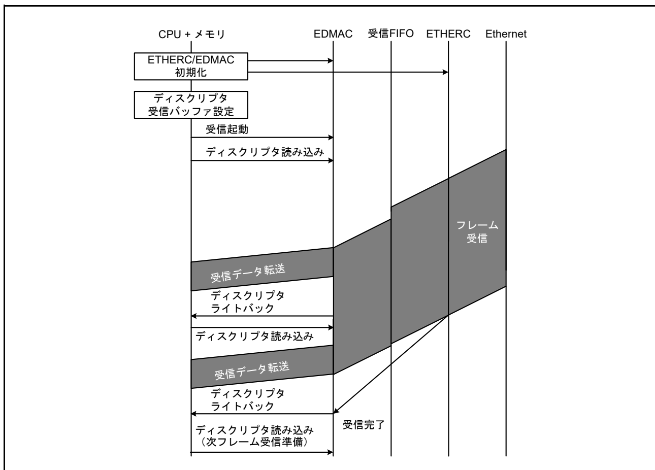
図 30.6 受信フローの例
