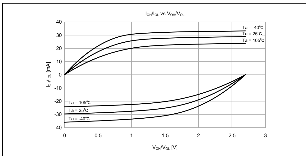
図 48.9 中駆動出力選択時の V_{CC} = 2.7V での V_{OH}/V_{OL} および I_{OH}/I_{OL} 温度特性（参考データ）
