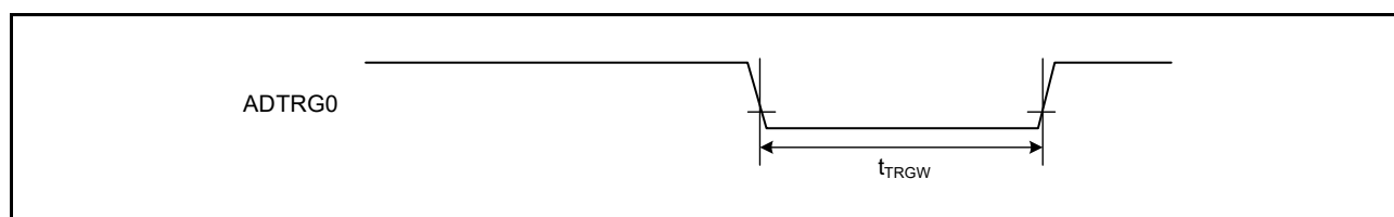
図 48.42 ADC14 トリガ入力タイミング
