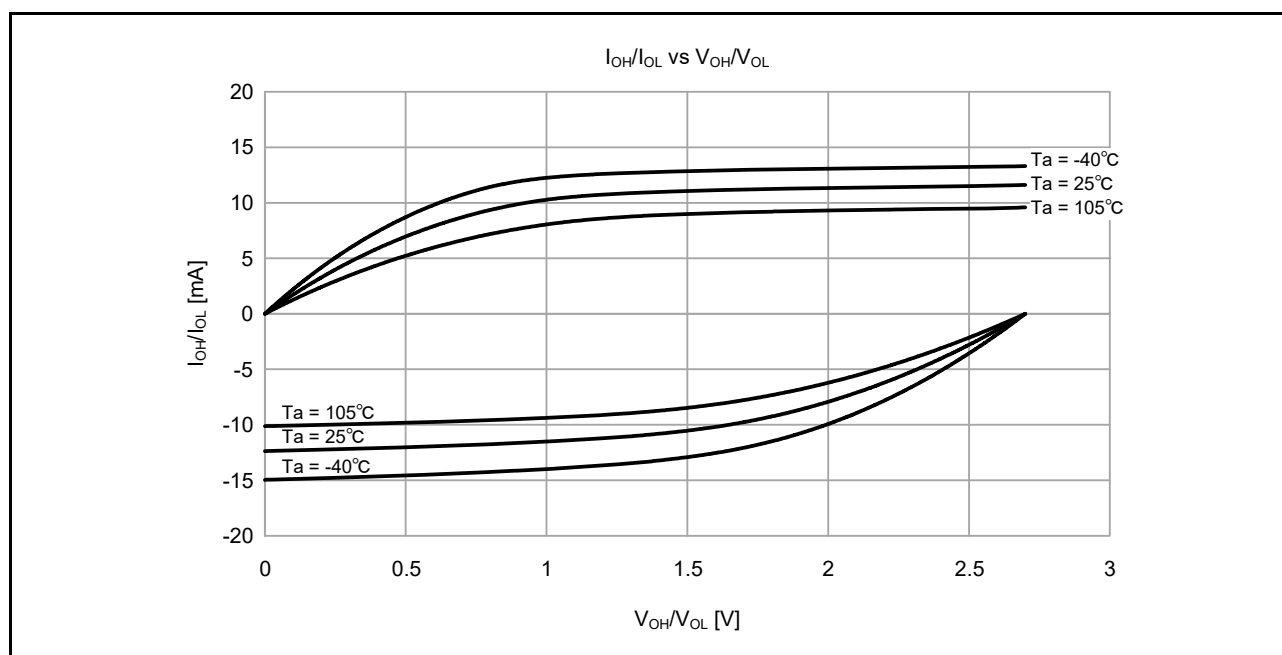
図 48.4 低駆動出力選択時の V_{CC} = 2.7\text{V} での V_{OH}/V_{OL} および I_{OH}/I_{OL} 温度特性 (参考データ)
