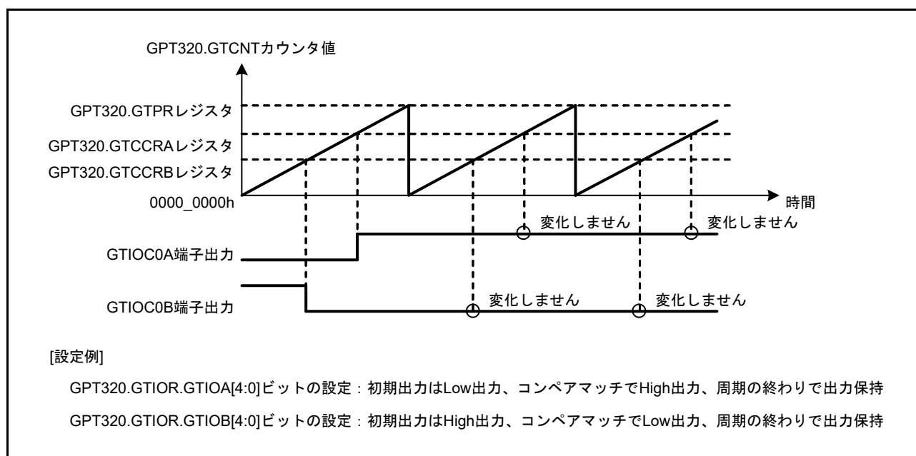
図 22.11 Low 出力／High 出力動作例
