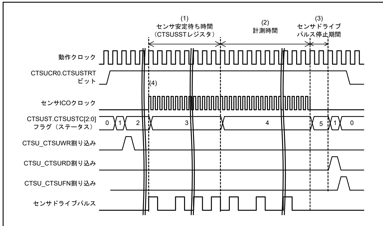
図 41.18 センサ安定待ちと計測のタイミング
