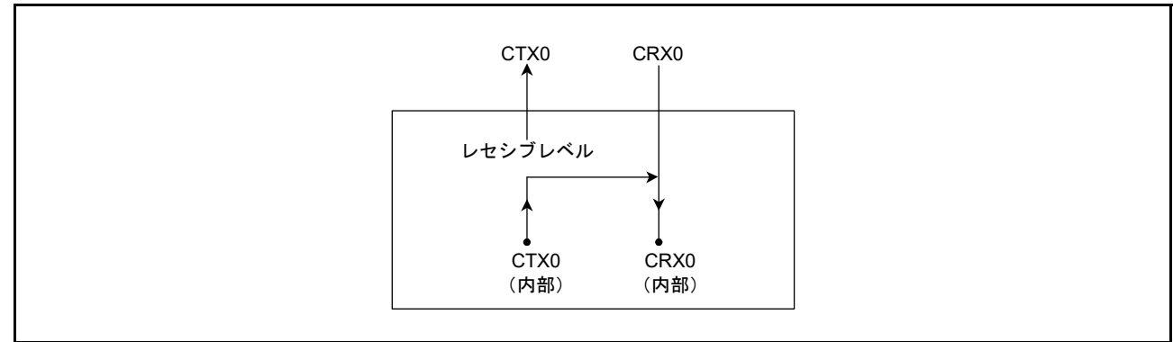
図 30.6 リッスンオンリモード選択時の接続
