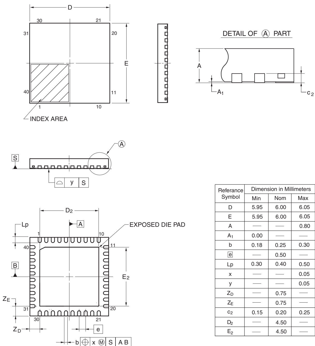
图 2.9 40-pin QFN (1)
