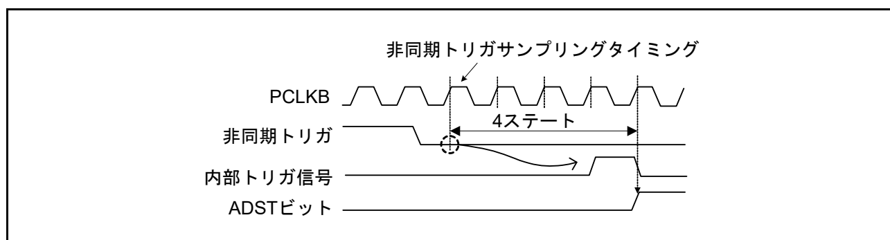
図 35.29 非同期トリガ入力タイミング
