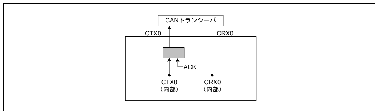
図 30.7 セルフテストモード 0 選択時の接続
