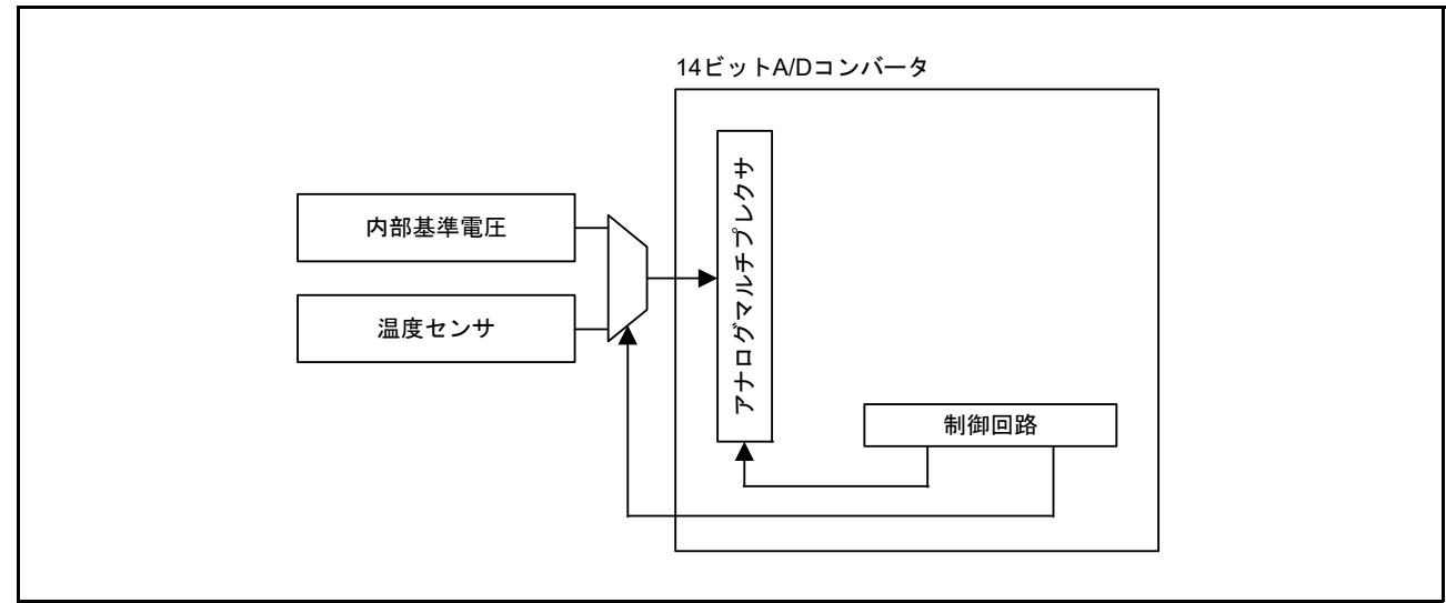
図 37.1 温度センサのブロック図
