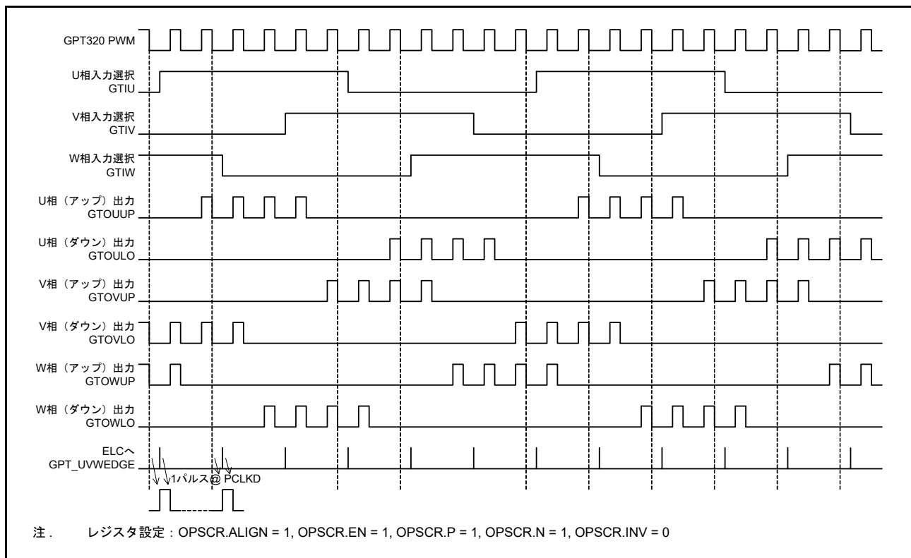
図 22.79 6 相 PWM 出力動作例 (チョップパ制御)
