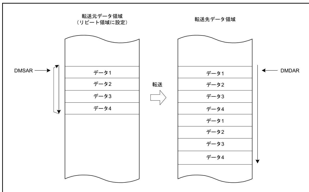
図 16.3 リピート転送モードにおける転送動作
