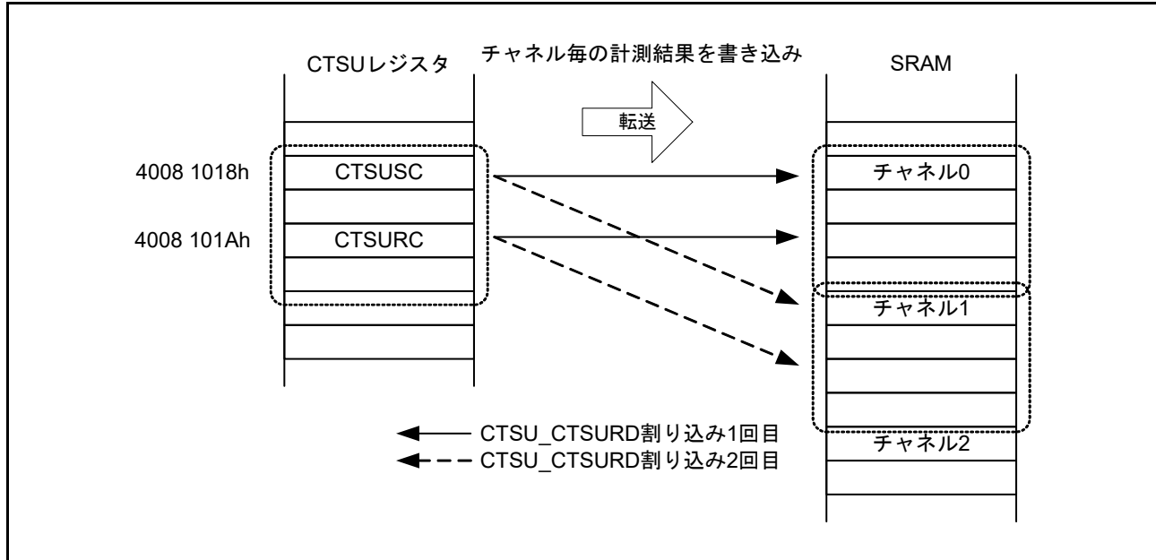
図 41.20 CTSUS_CTSURD 割り込みを用いた DTC 転送動作例
