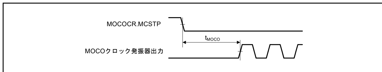
図 48.31 MOCO クロック発振開始タイミング
