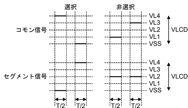
(f) 1/4バイアス法 (B波形)
