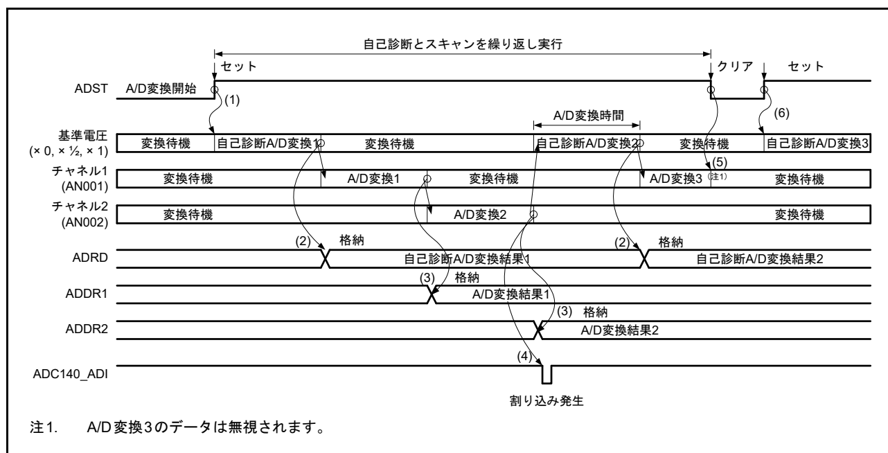
図 35.12 連続スキャンモードの基本動作例 (AN001 および AN002 選択 + 自己診断)
