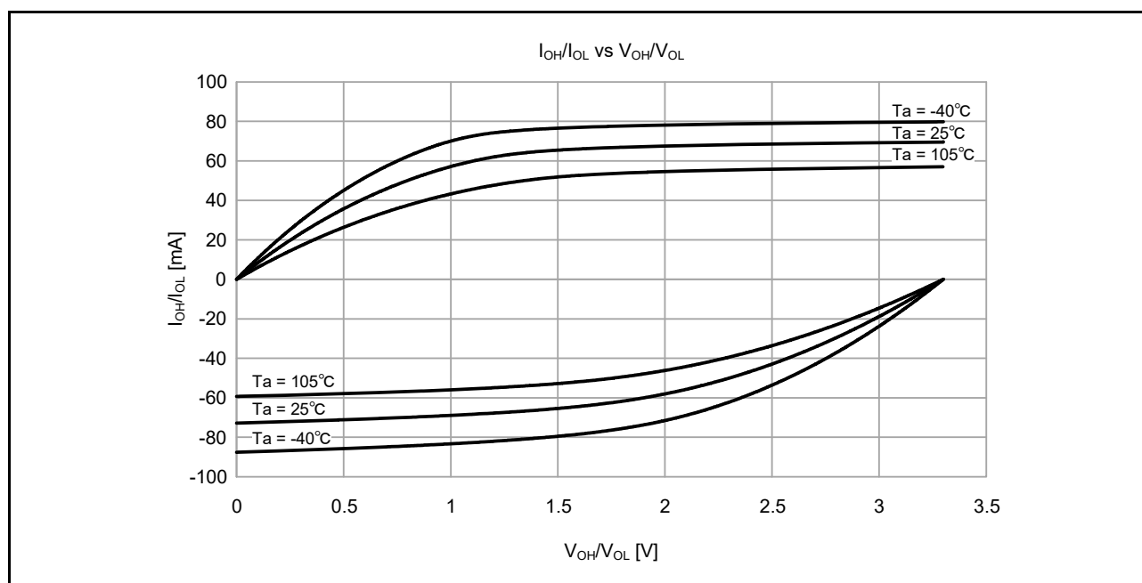
図 48.14 中駆動出力選択時の V_{CC} = 3.3V での V_{OH}/V_{OL} および I_{OH}/I_{OL} 温度特性 (参考データ)
