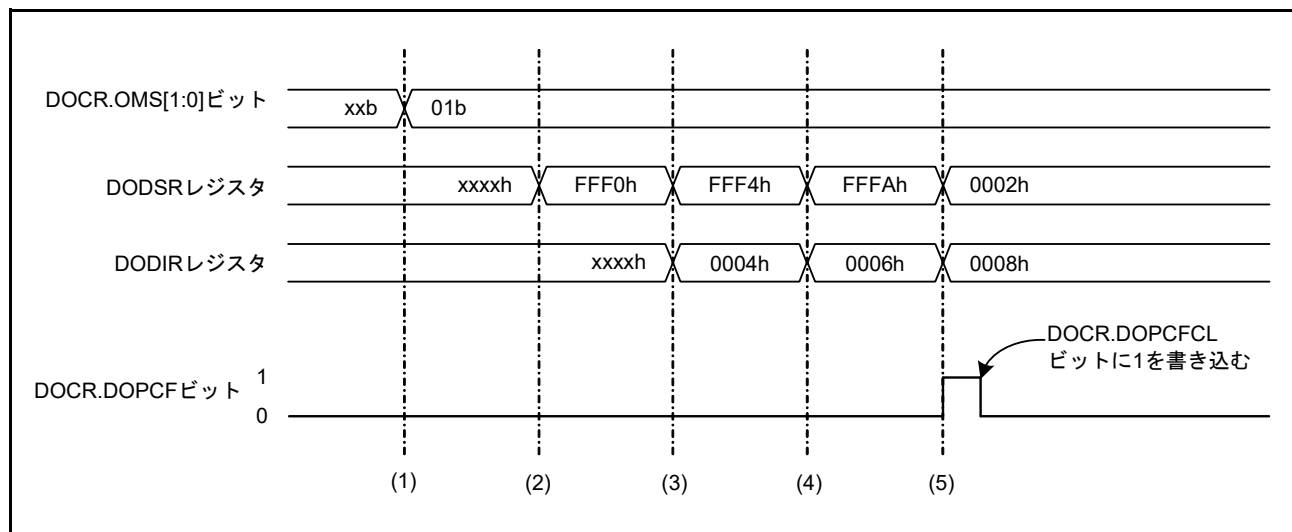
図 42.3 データ加算モードの動作例
