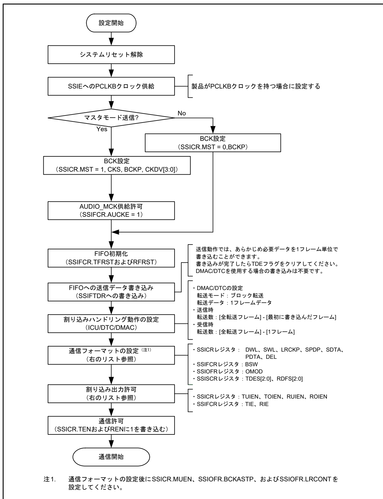
図 33.49 通信開始手順 (CPU 動作手順)
