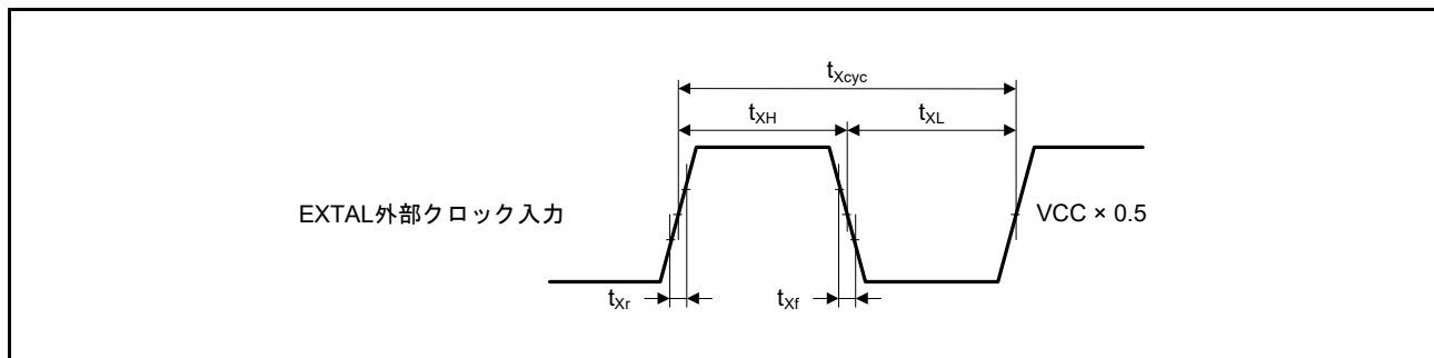
図 48.25 EXTAL 外部クロック入力タイミング
