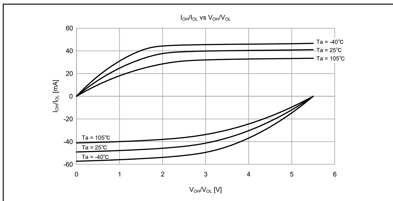
図 48.6 低駆動出力選択時の V_{CC} = 5.5\text{V} での V_{OH}/V_{OL} および I_{OH}/I_{OL} 温度特性 (参考データ)
