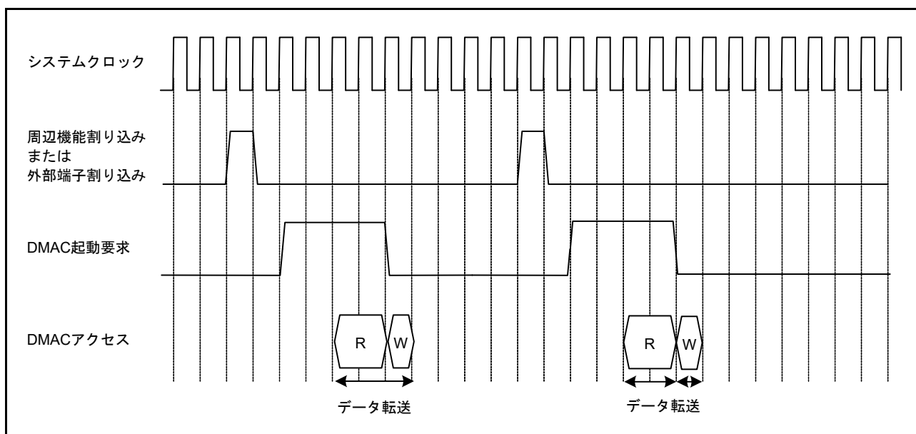
図 16.10 DMAC 動作タイミング例 1 (ノーマル転送モードまたはリポート転送モードでの周辺モジュールまたは外部割り込み入力端子からの割り込みによる DMA 起動)
