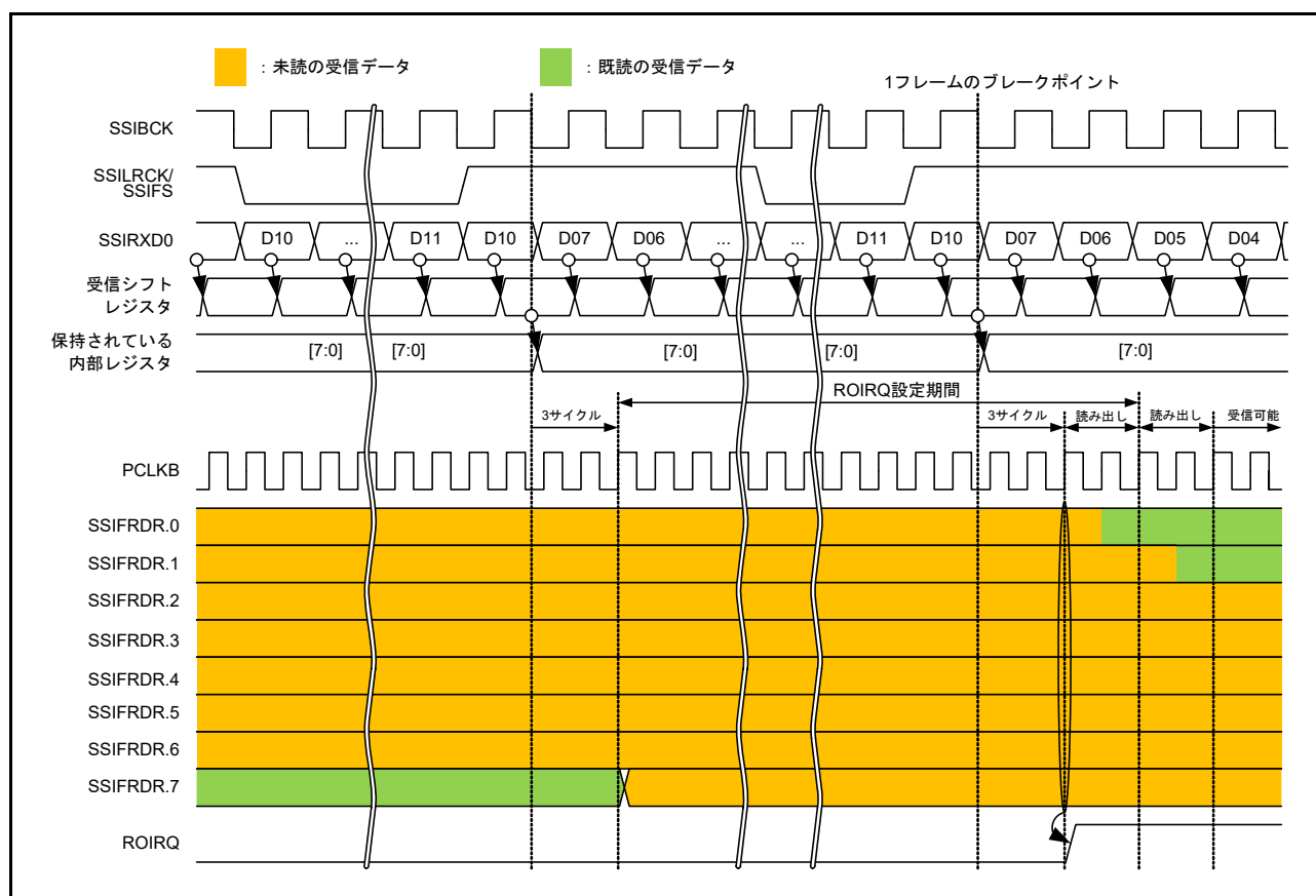
図 33.14 ROIRQ 設定タイミング
