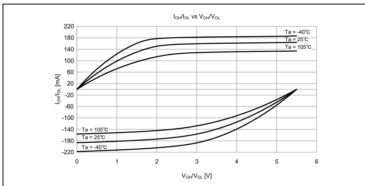
図 48.15 中駆動出力選択時の V_{CC} = 5.5V での V_{OH}/V_{OL} および I_{OH}/I_{OL} 温度特性 (参考データ)
