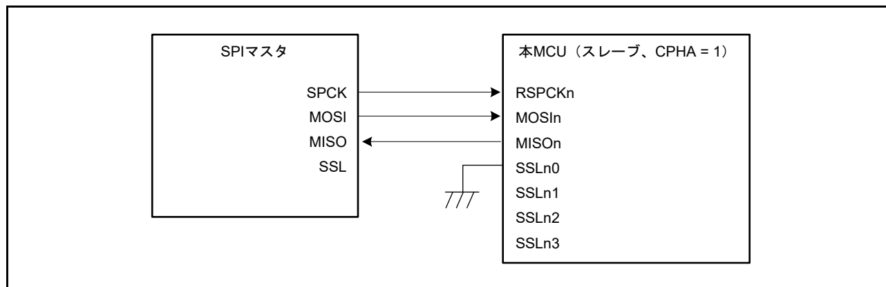
図 31.7 シングルマスタとシングルスレーブの構成例 (MCU はスレーブ、CPHA = 1)
