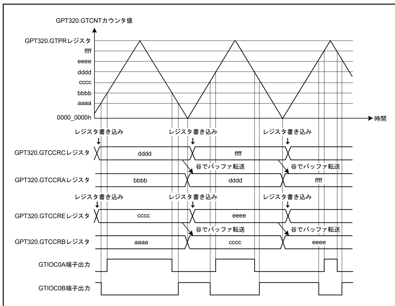
図 22.33 三角波 PWM モード 1 動作例 (バッファ動作、カウントスタート時 GTIOCA 端子 = Low 出力 / GTIOCB 端子 = High 出力、GTCCR A/GTCCR B レジスタのコンペアマッチでトグル出力、周期の終わりで出力保持の場合)
