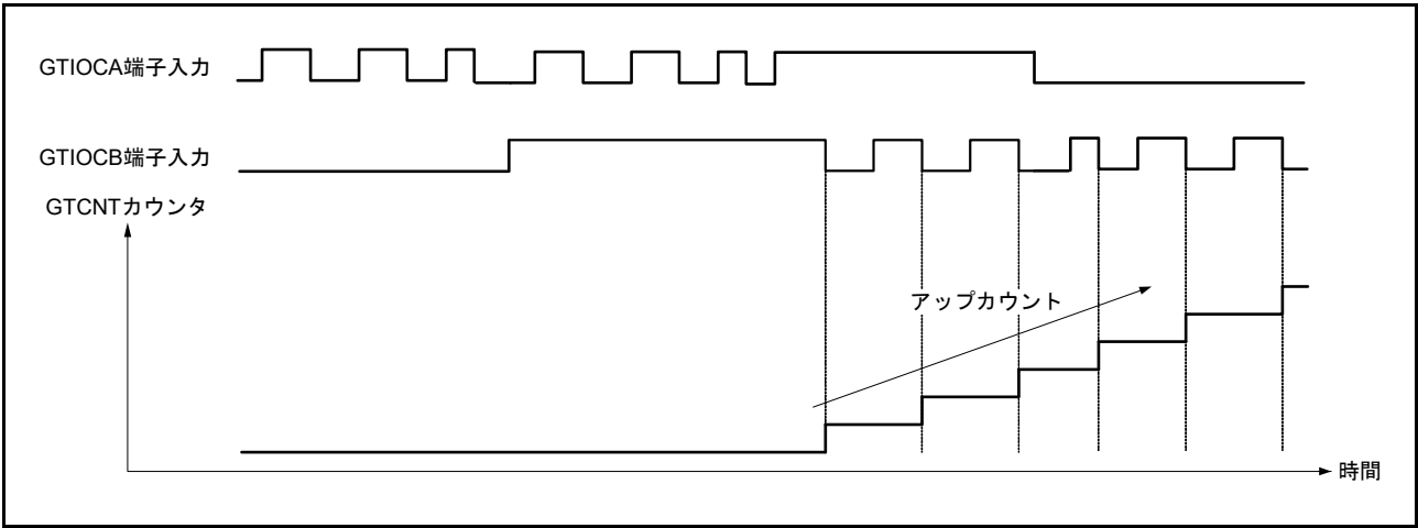
図 22.76 位相計数モード 5 動作例 (B)
