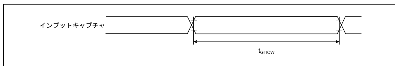
図 48.40 GPT インพุットキャプチャタイミング
