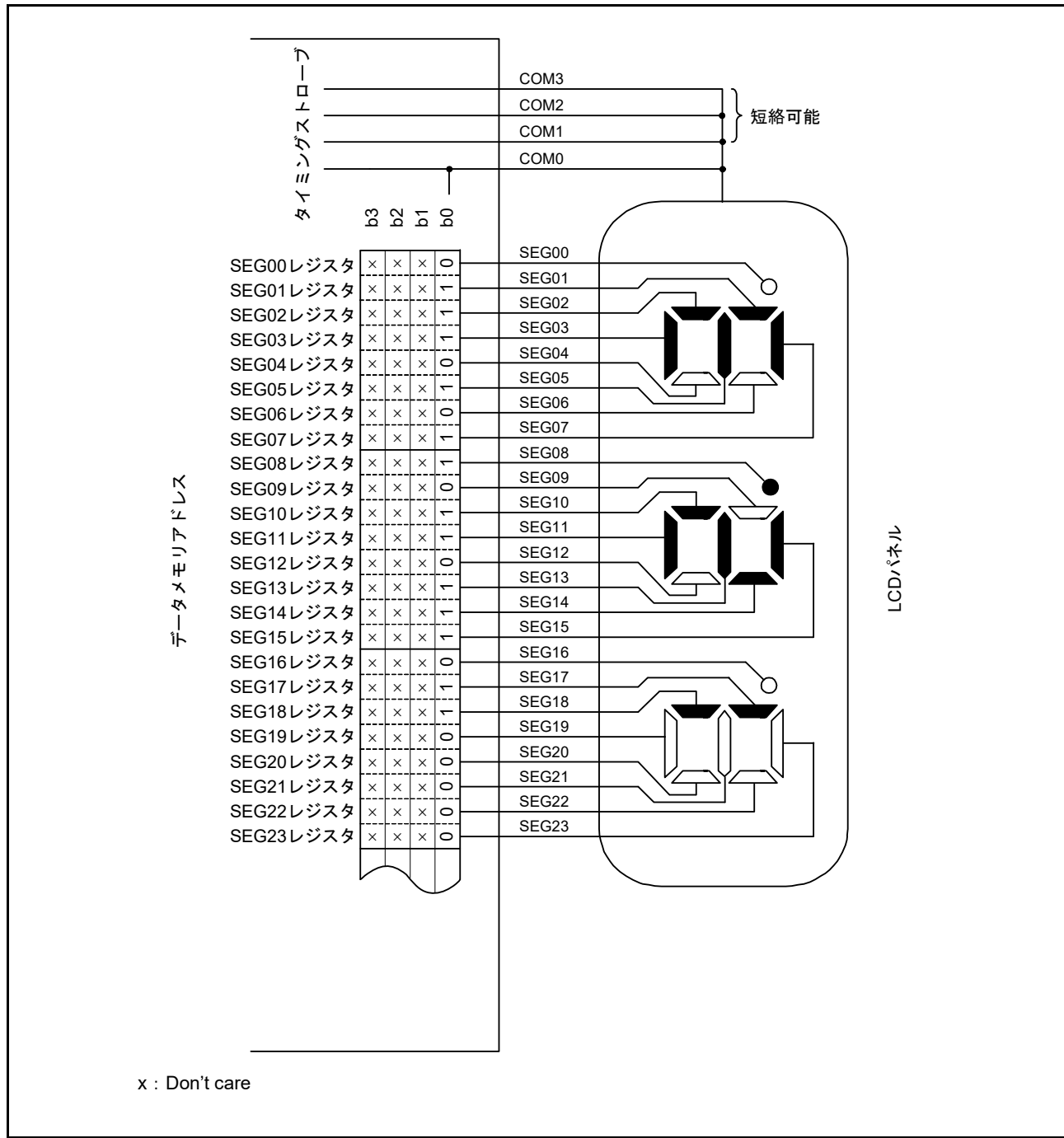
図 45.19 スタティック LCD パネルの接続例
