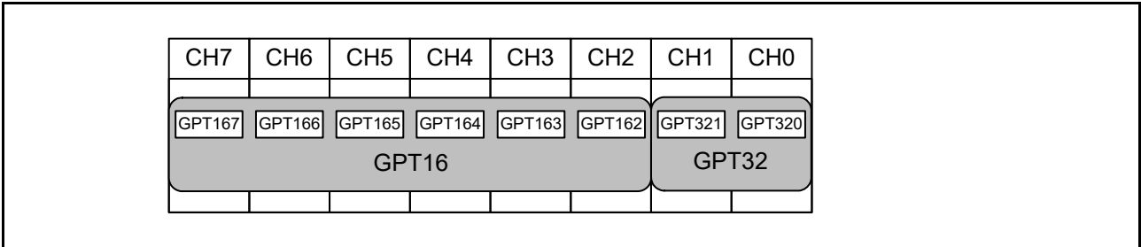
図 22.2 GPT チャンネルとモジュール名の対応関係
