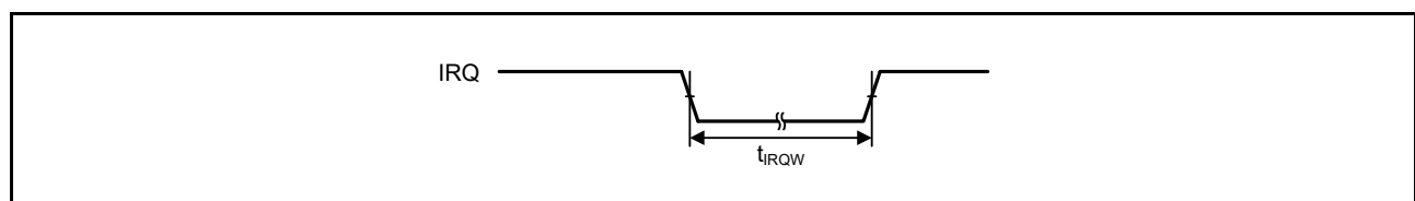
図 48.37 IRQ 割り込み入力タイミング
