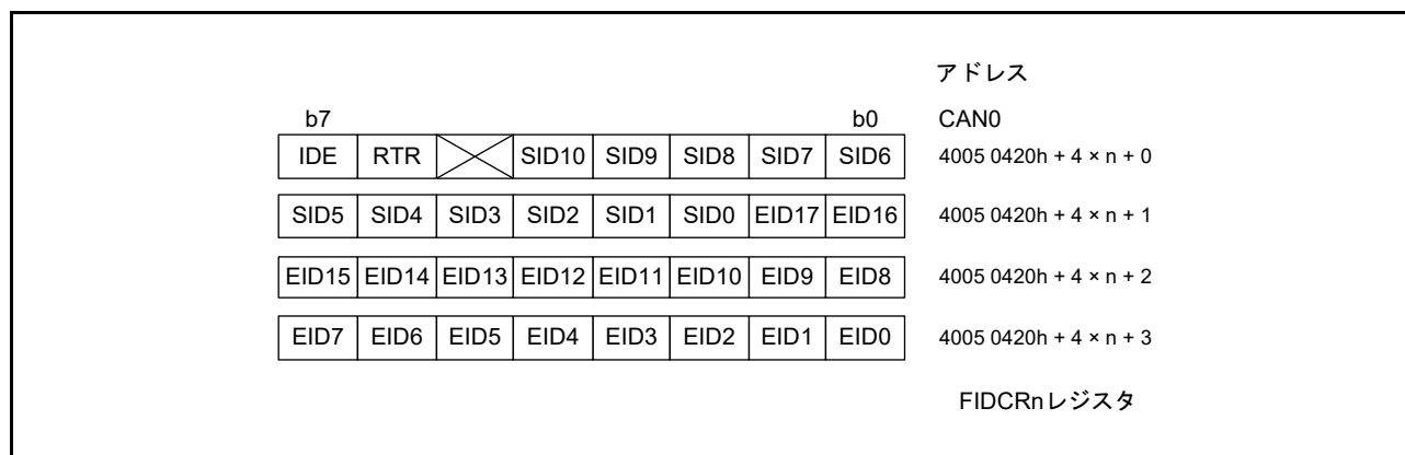
図 30.15 FIDCRn レジスタの構成 (n = 0, 1)
