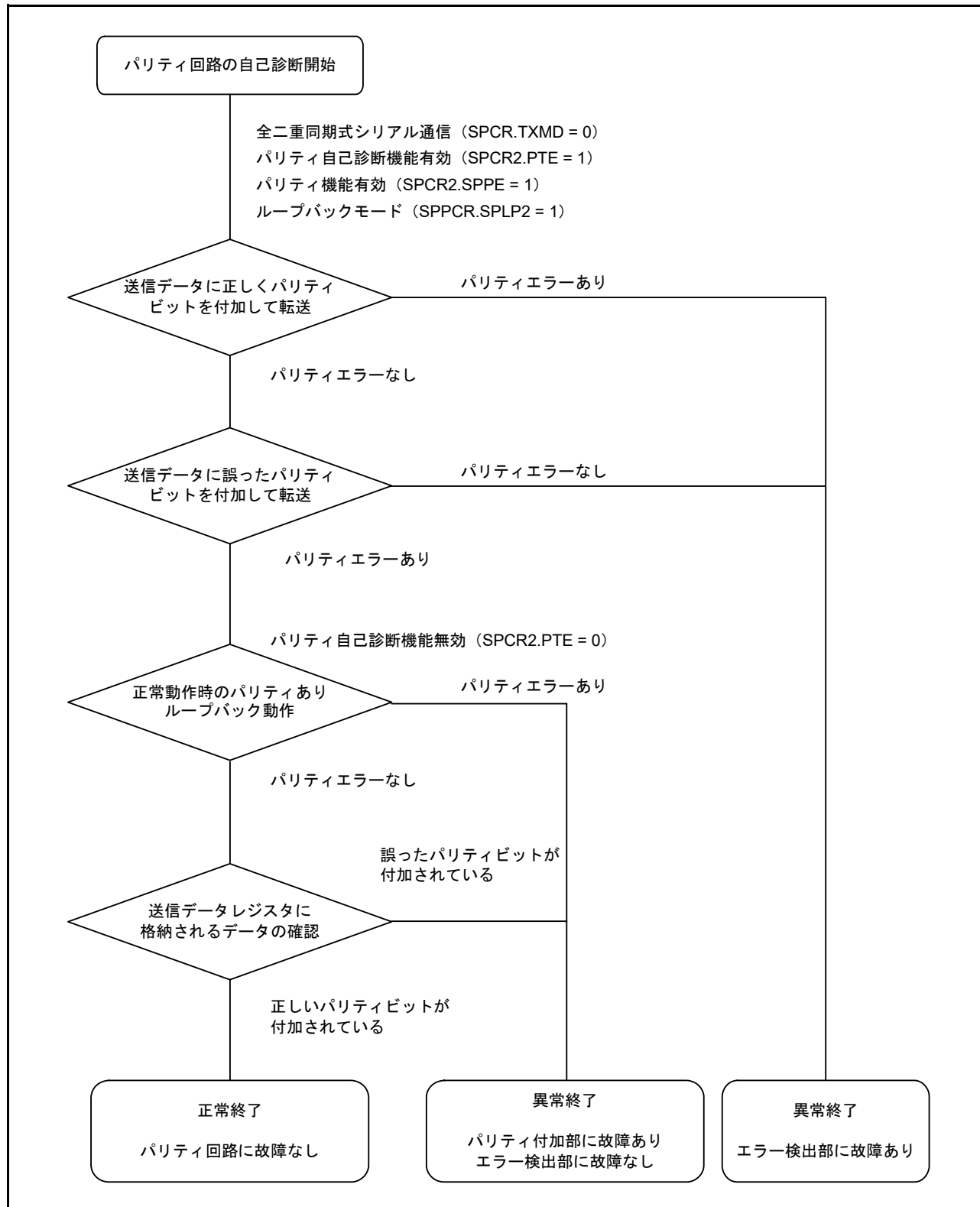
図 31.43 パリティ回路の自己診断フロー
