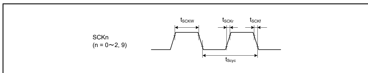
図 48.44 SCK クロック入力タイミング
