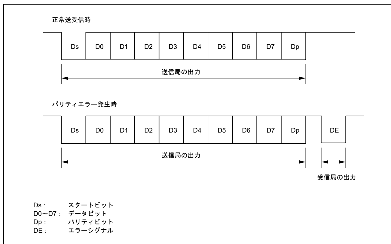
図 28.46 スマートカードインタフェースモードにおけるデータフォーマット
