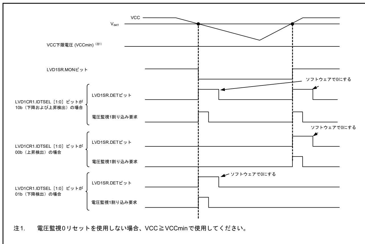
図 7.5 電圧監視 1 割り込みの動作例
