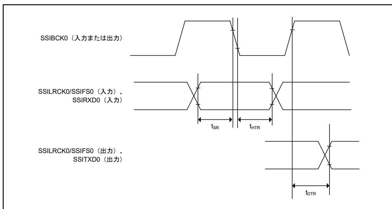
図 48.62 SSIE データ送受信タイミング (SSICR.BCKP = 1)
