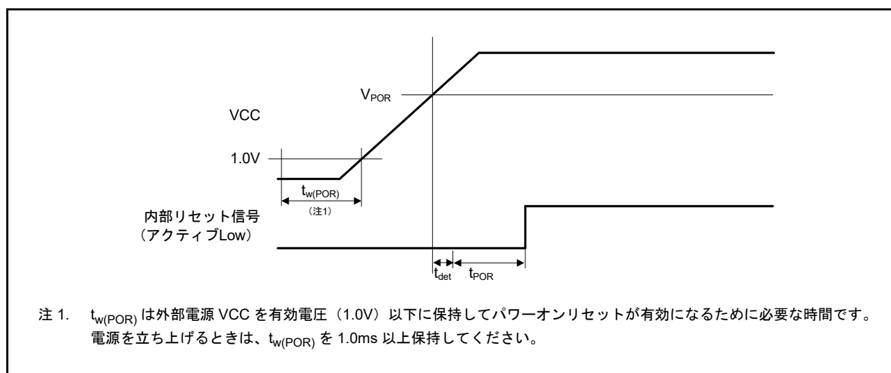
図 48.74 パワーオンリセットタイミング
