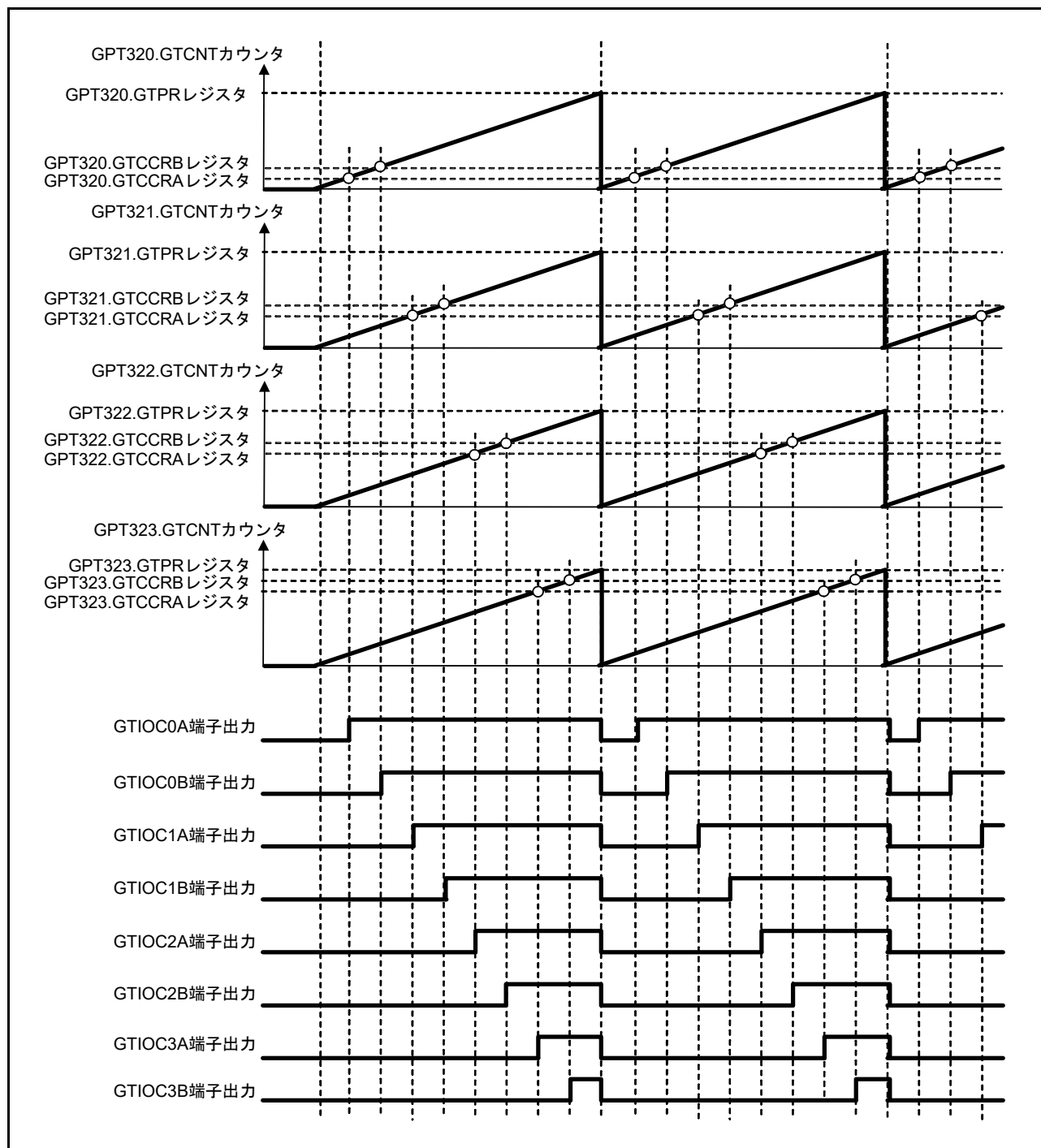
図 22.61 同期 PWM 出力例
