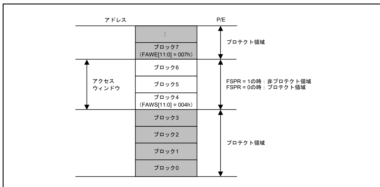
図 6.2 アクセスウィンドウの概要
