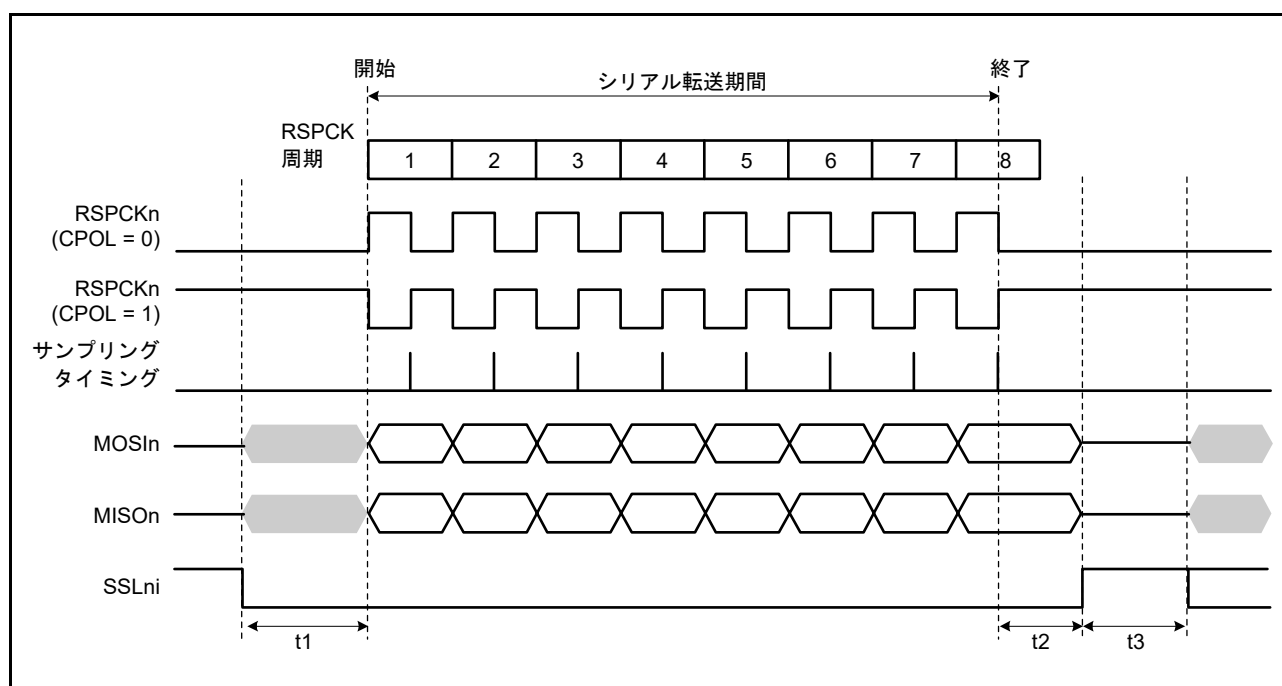
図 31.23 SPI 転送フォーマット (CPHA ビット = 1)
