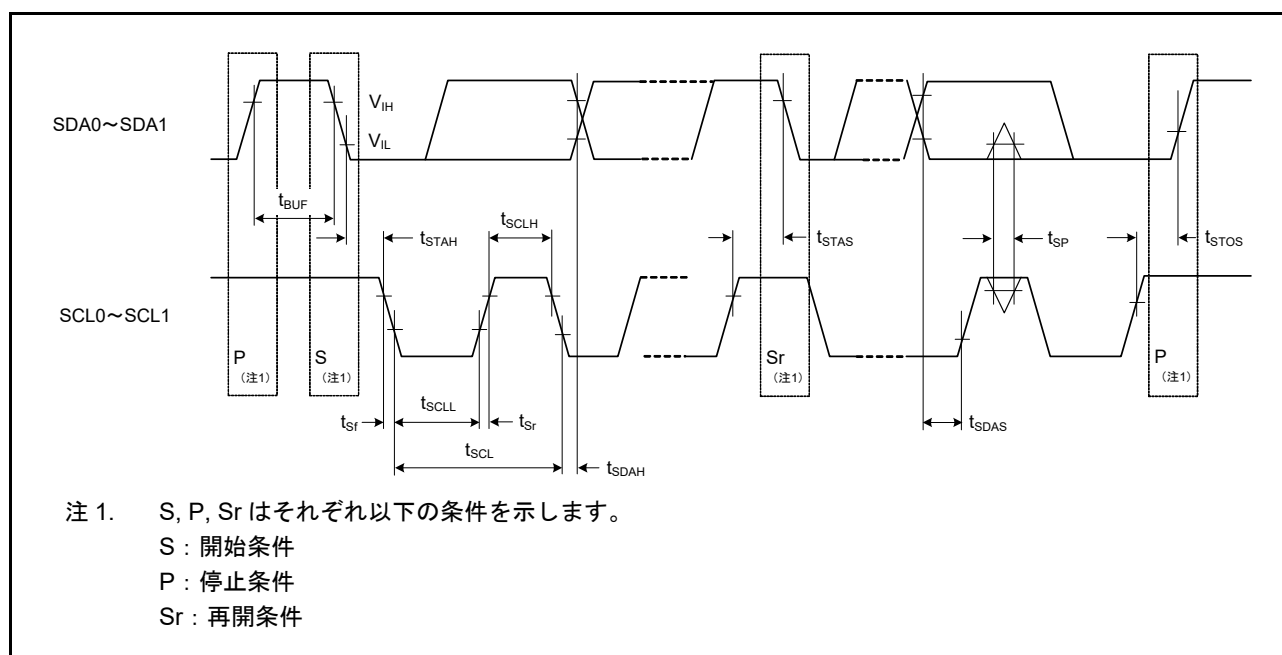
図 48.59 IIC バスインタフェース入出力タイミング
