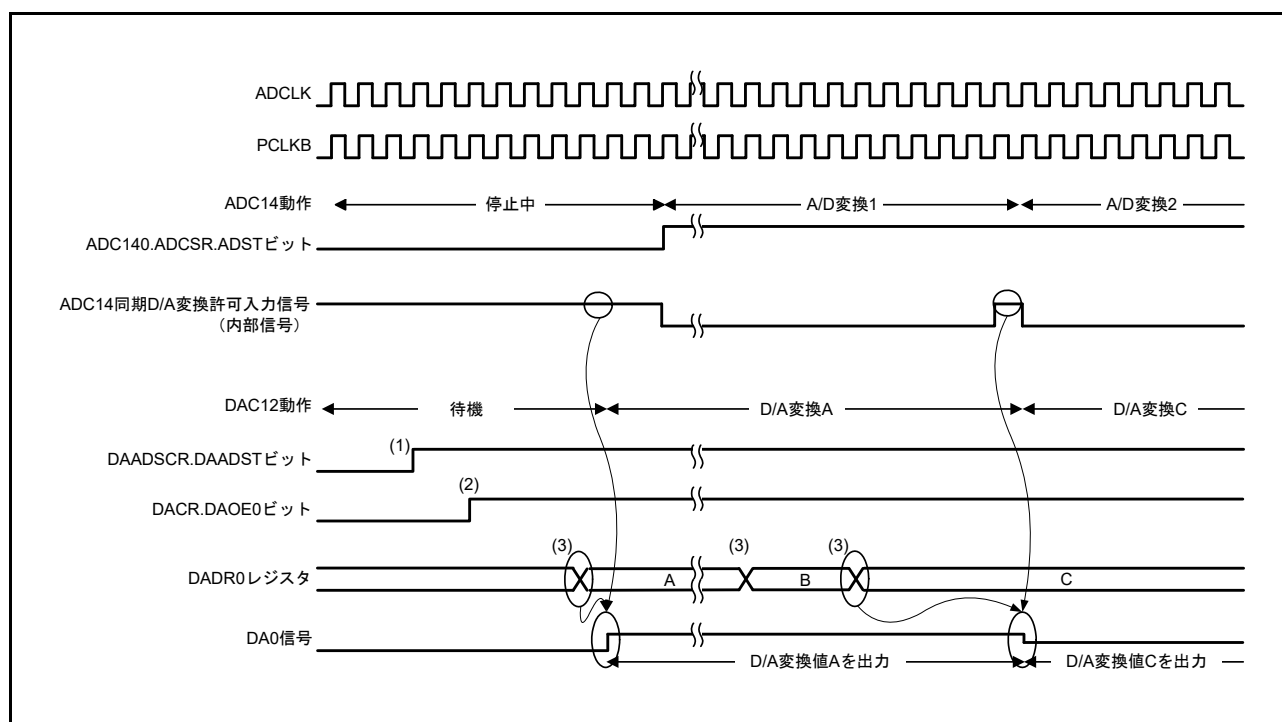
図 36.3 DAC12 を ADC14 に同期して変換する例
