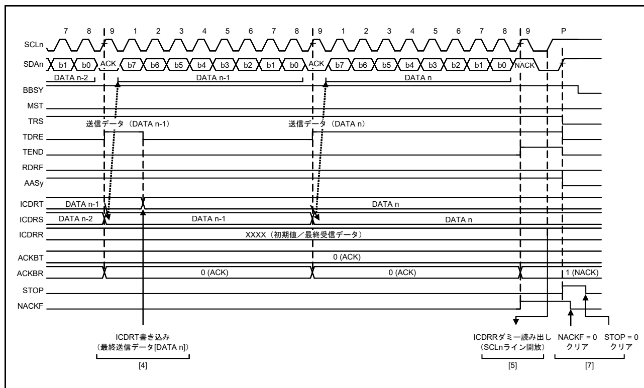
図 29.17 スレーブ送信の動作タイミング (2)
