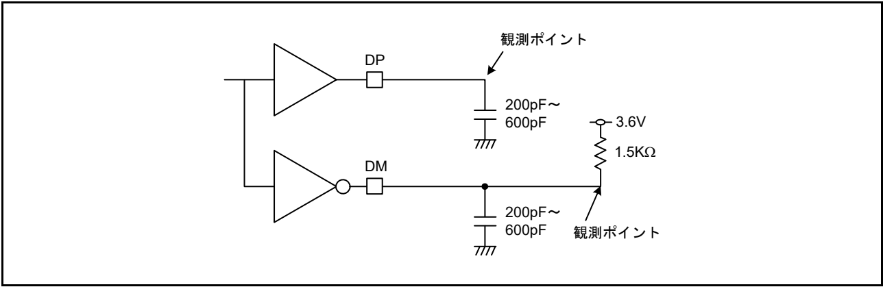
図 48.67 ロースピード（LS）接続の測定回路
