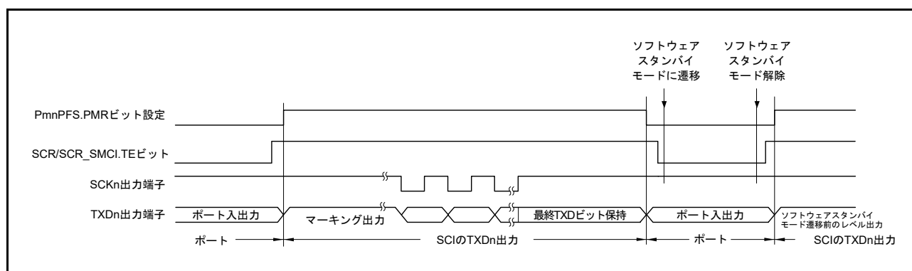
図 28.75 ソフトウェアスタンバイモード遷移中のポートの端子状態 (内部クロック、クロック同期送信)
