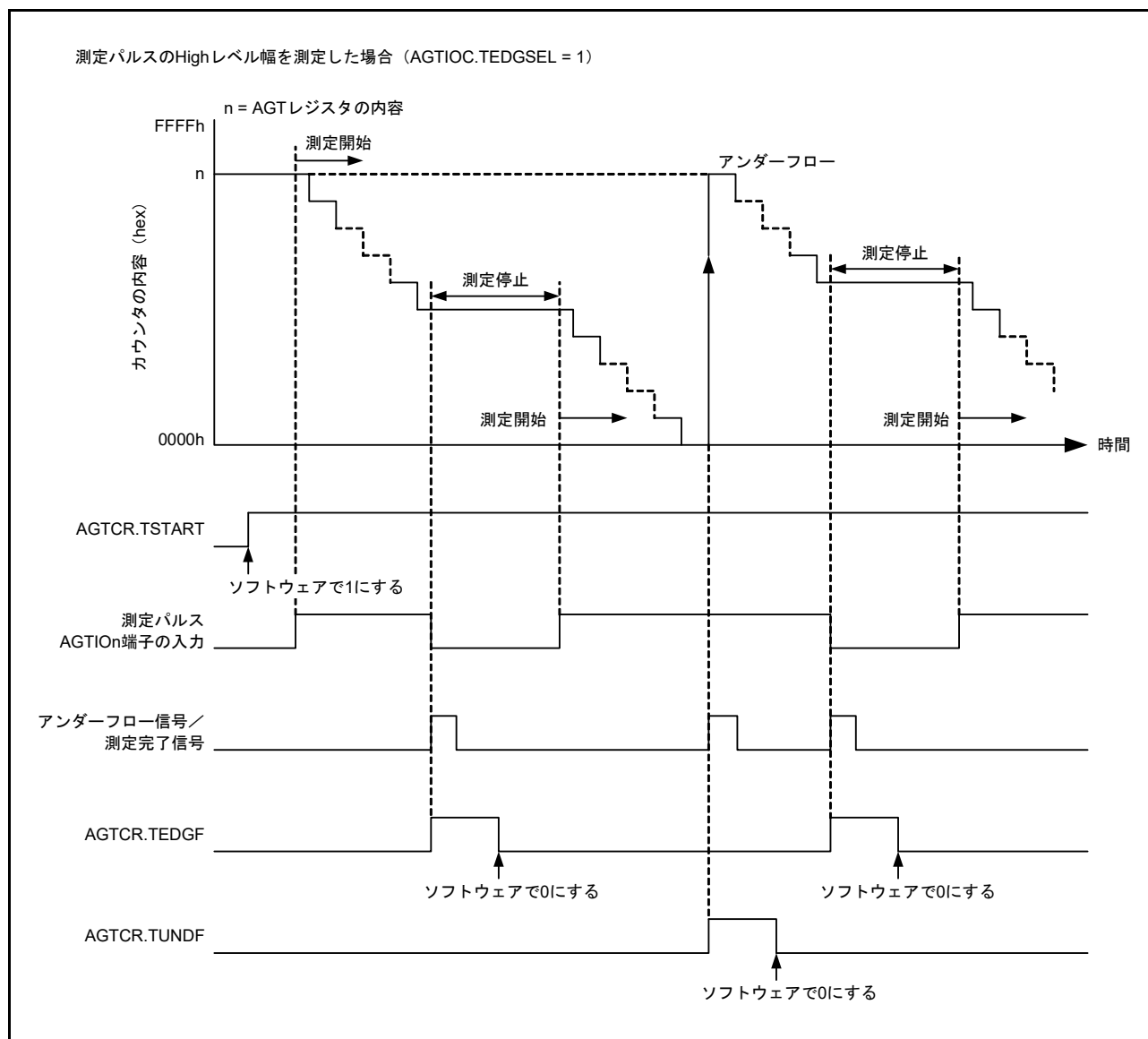
図 23.9 パルス幅測定モードでの動作例
