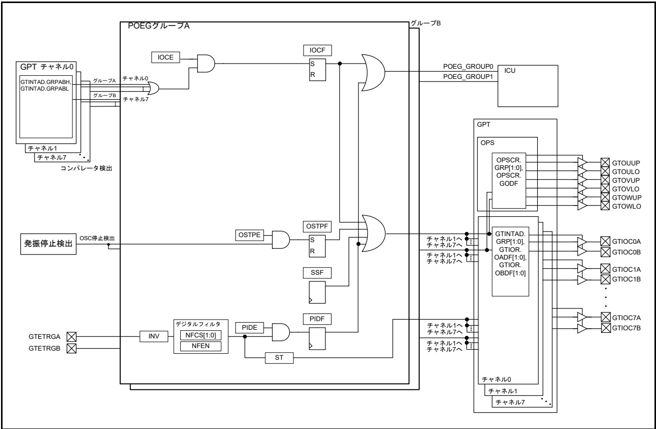
図 21.1 POEG のブロック図
