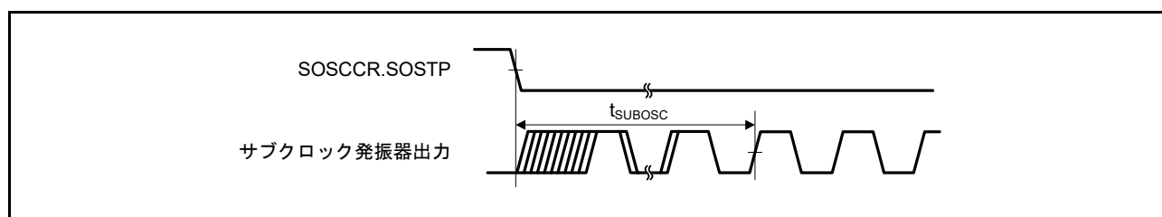
図 48.30 サブクロック発振開始タイミング
