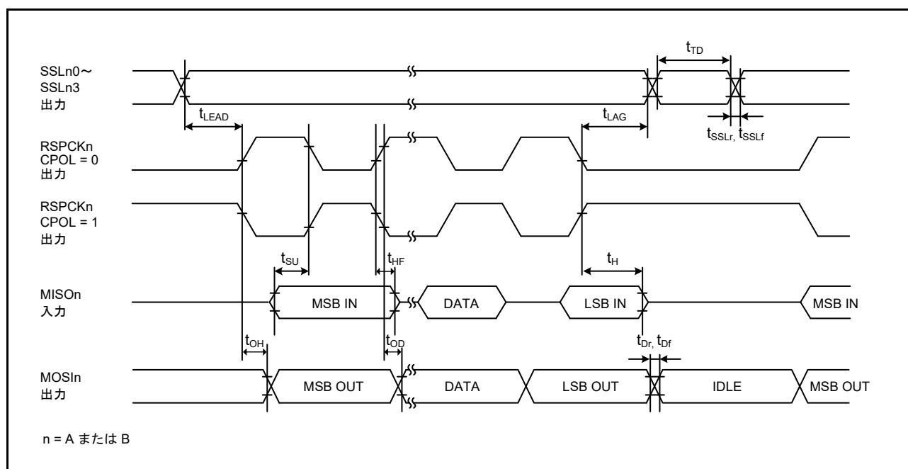
図 48.56 SPI タイミング (マスタ、CPHA = 1) (ビットレート : PCLKA を 2 分周に設定)
