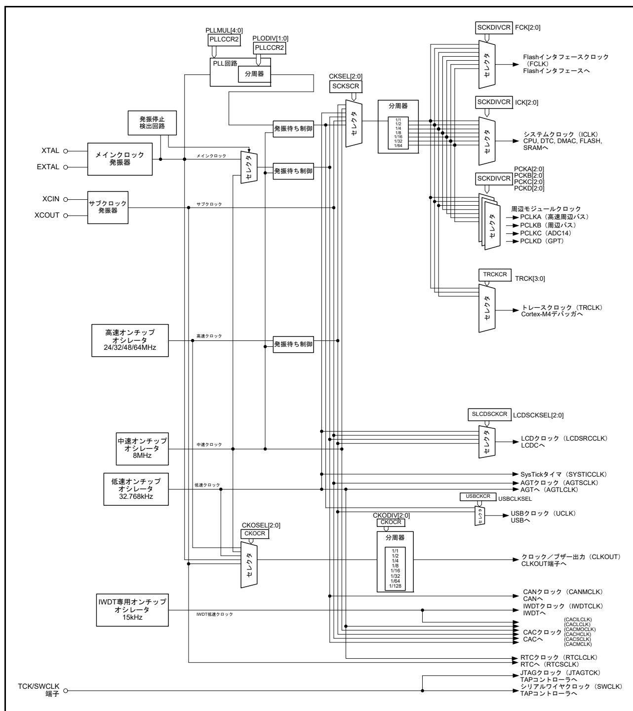
図 8.1 クロック発生回路のブロック図
