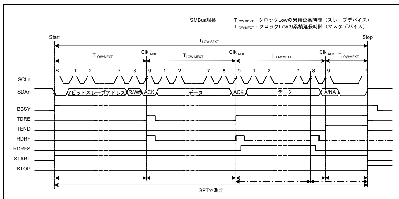
図 29.50 SMBus タイムアウト測定
