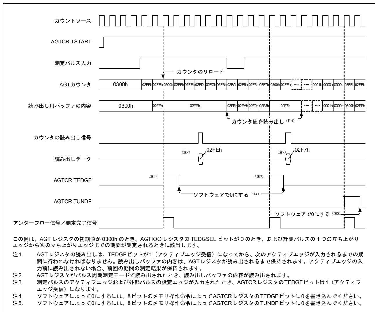
図 23.10 パルス周期測定モードでの動作例
