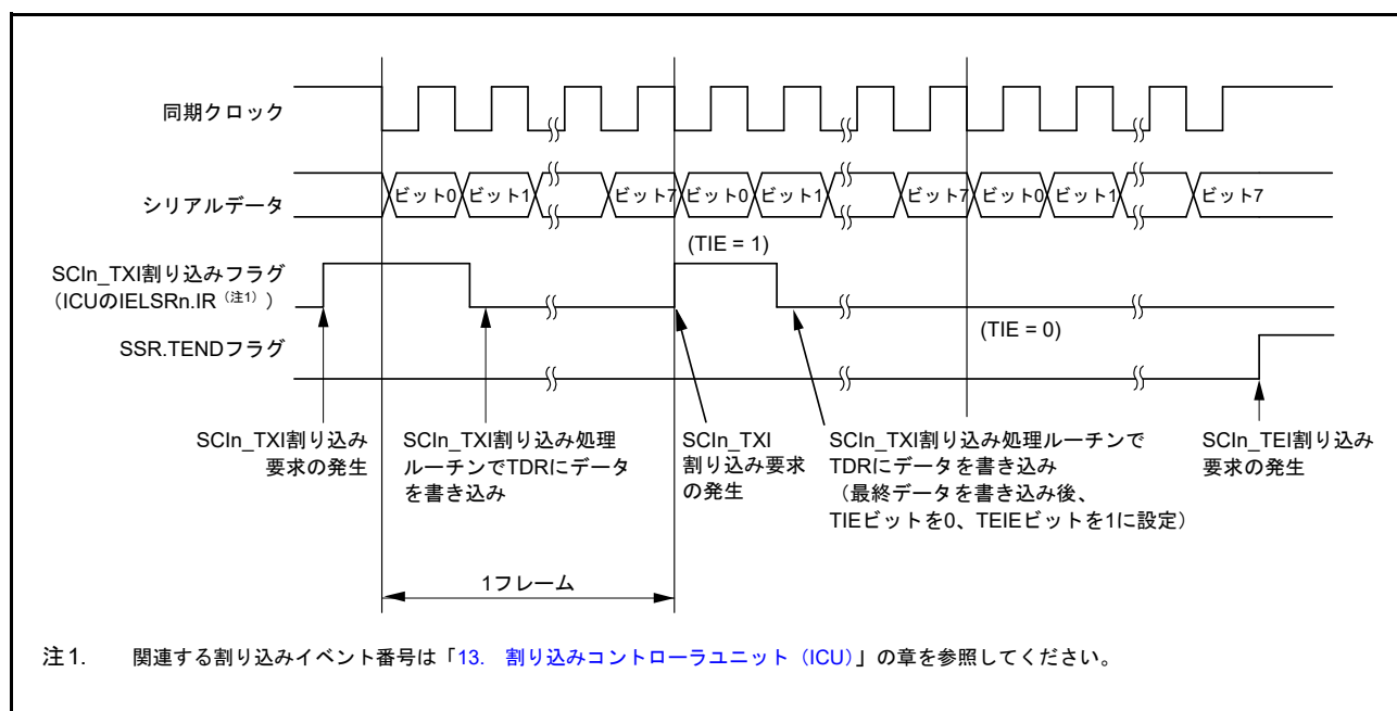
図 28.36 クロック同期式モードにおけるシリアル送信の動作例 (送信中～送信終了時)
