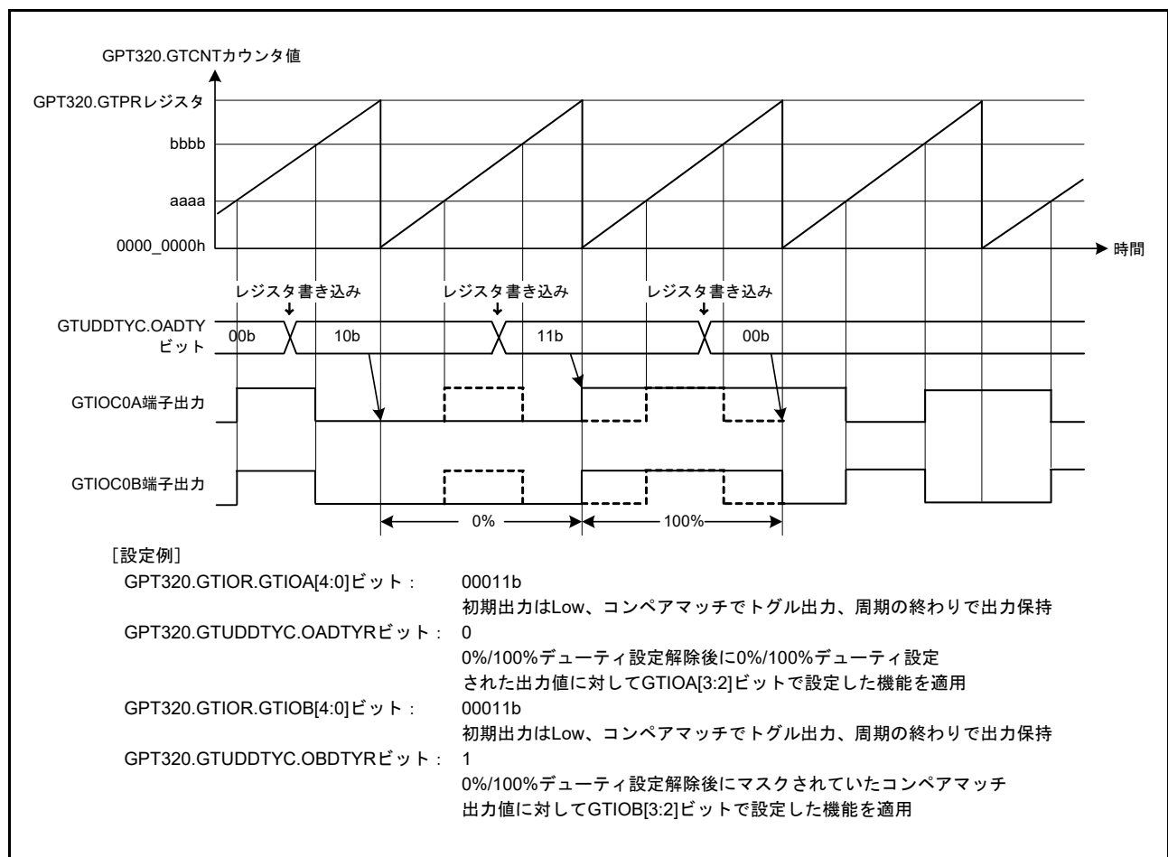
図 22.46 出力デューティ 0%、100% 機能動作例
