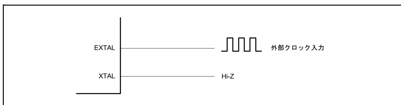
図 8.5 外部クロックの等価回路
