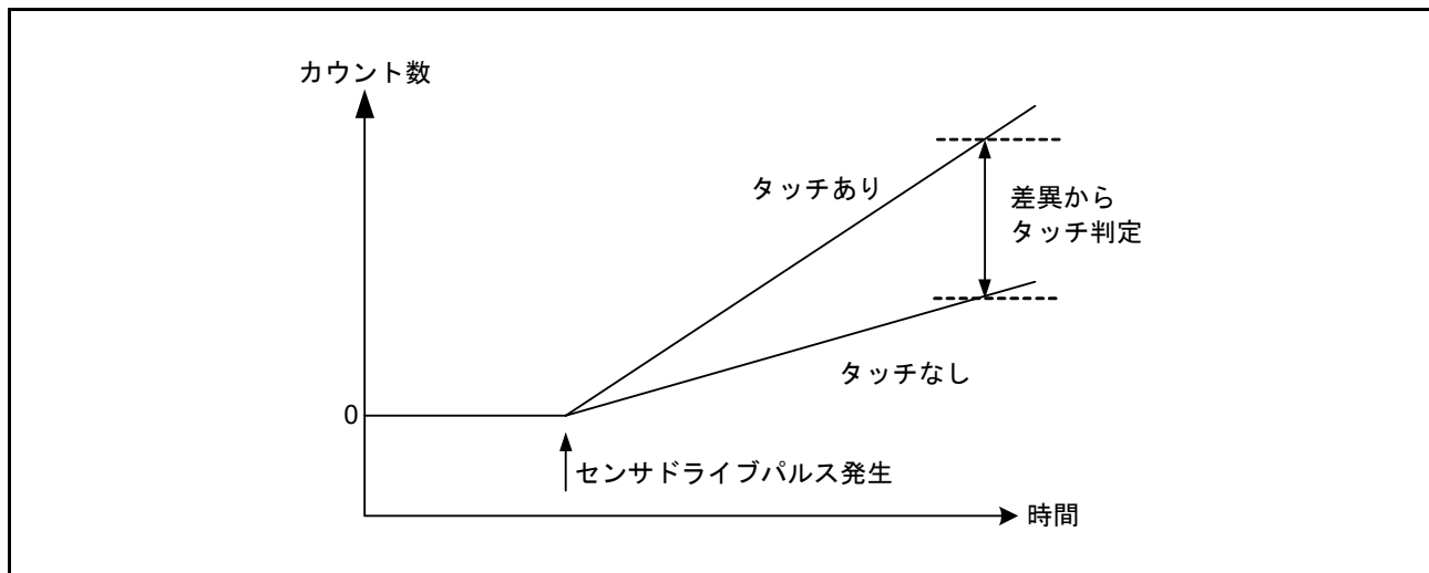
図 41.7 接触／非接触による計測値の変化
