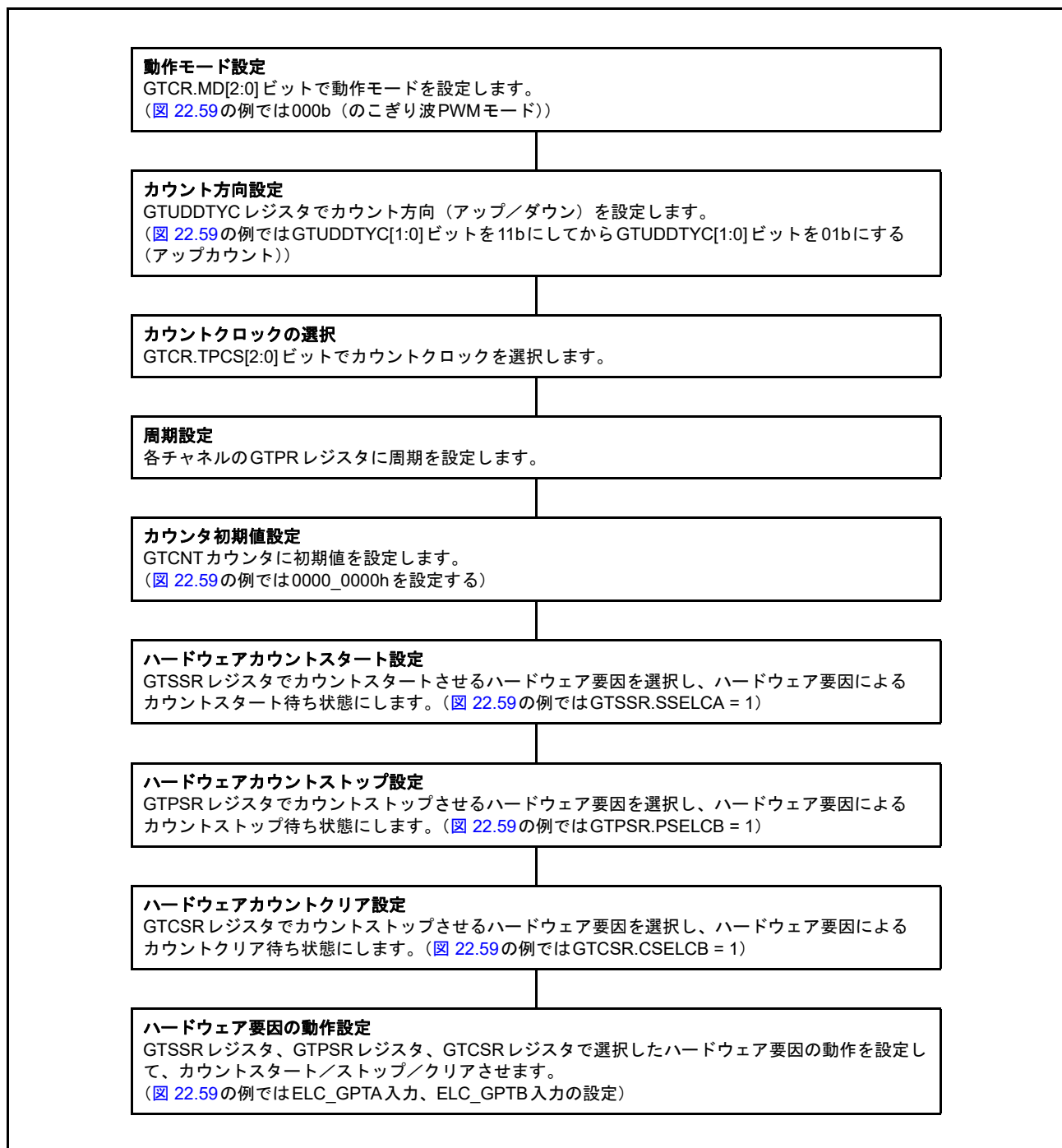
図 22.60 ハードウェア要因による同時スタート設定例
