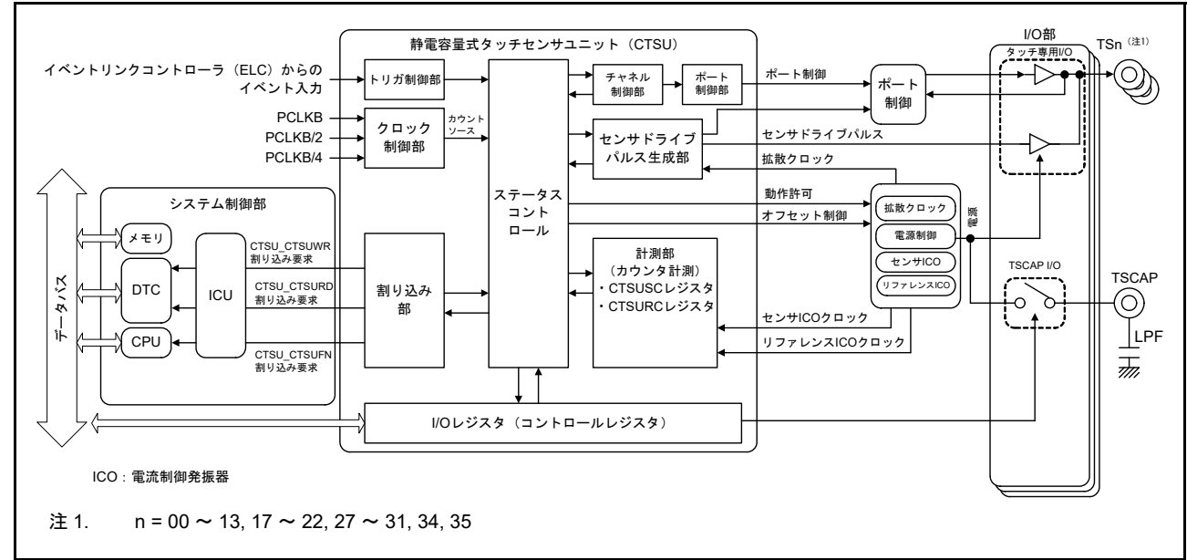
図 41.3 CTSU のブロック図
