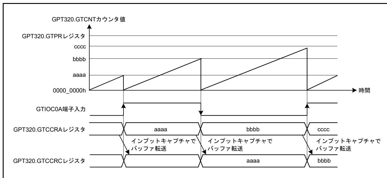
図 22.26 GTCCRA、GTCCRB レジスタのバッファ動作例 (GTIOC0A 端子入力の両エッジでインプットキャプチャ、のこぎり波でアップカウント、GTIOC0A 端子入力の両エッジで GTCNT カウンタクリアの場合)
