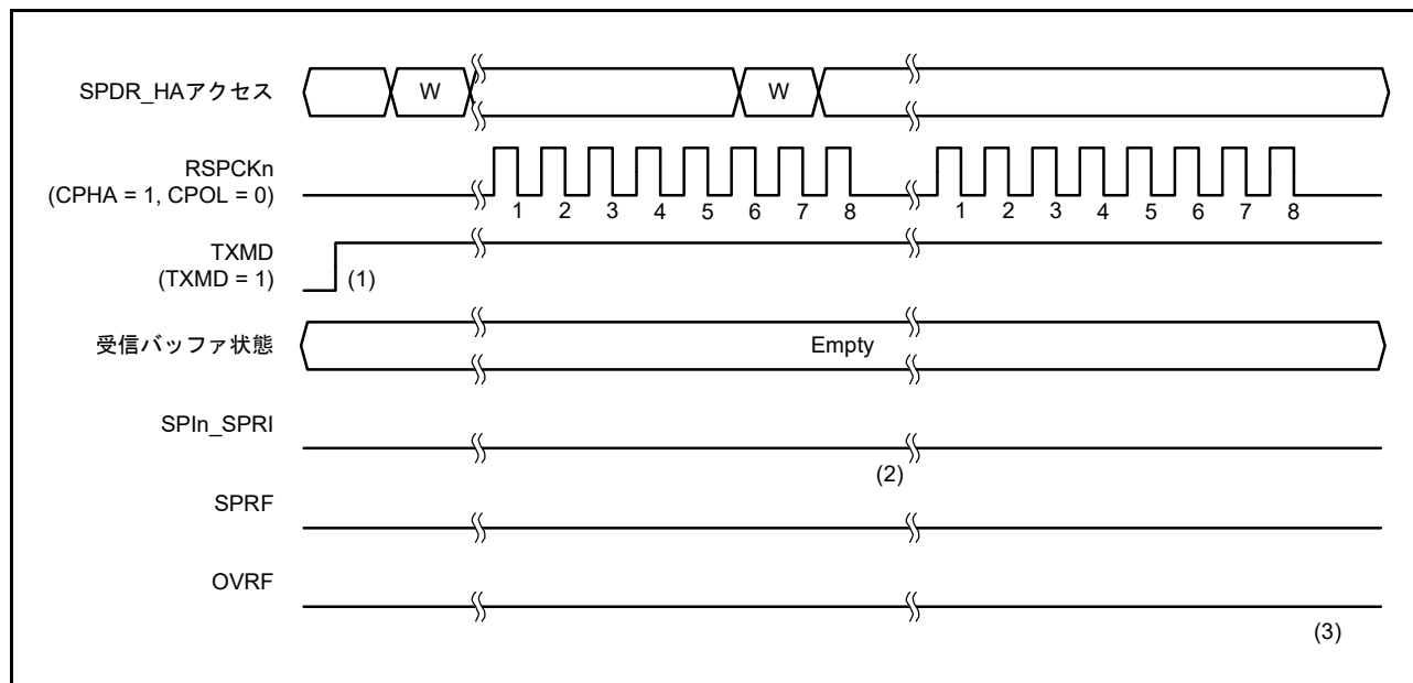
図 31.25 SPCR.TXMD = 1 の動作例
