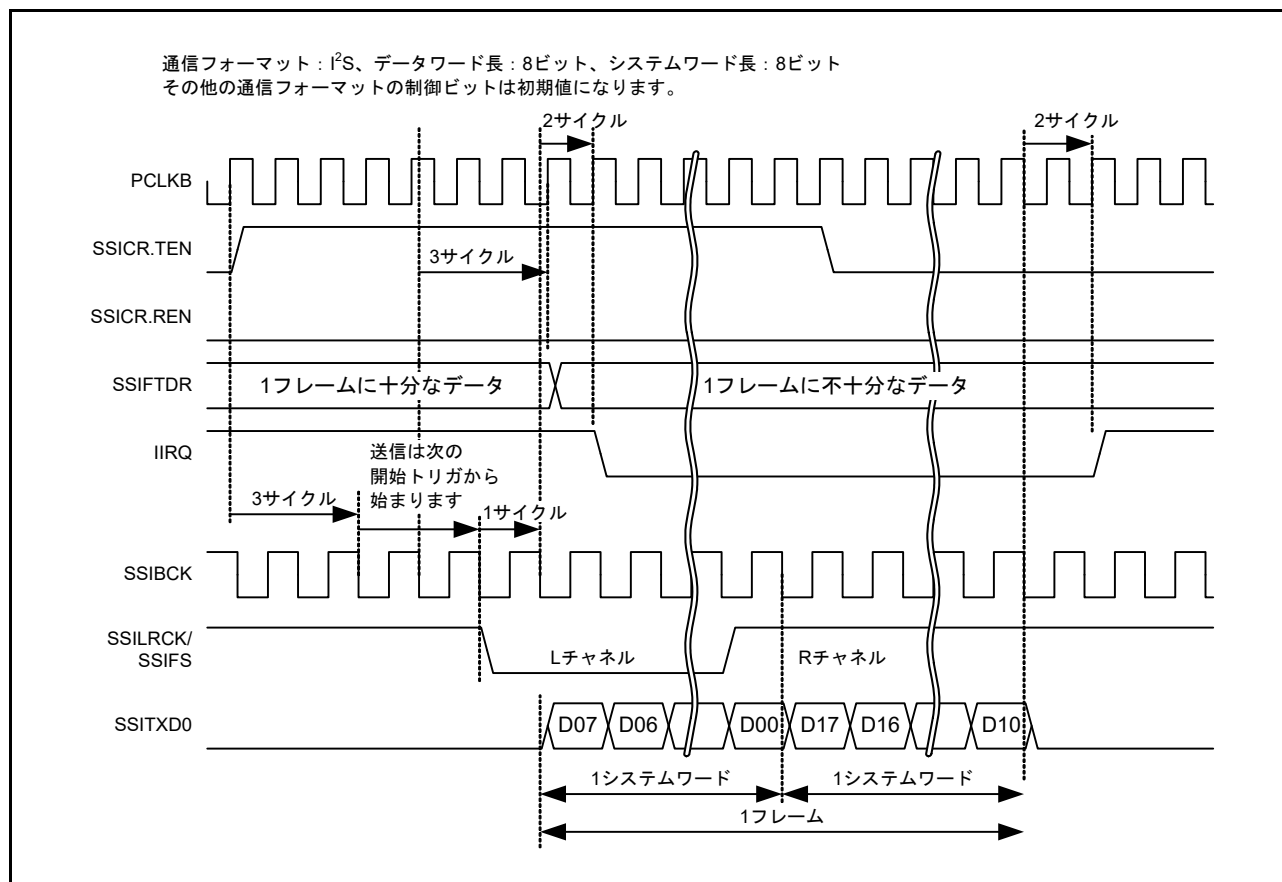
図 33.12 IIRQ 設定タイミング (送信)
