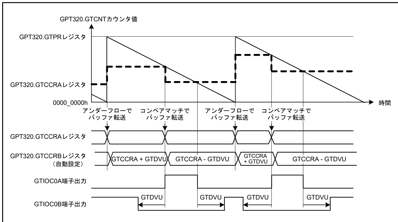
図 22.40 デッドタイム自動設定機能の動作例（のこぎり波ワンショットパルスモード、ダウンカウント、アクティブ High の場合）
