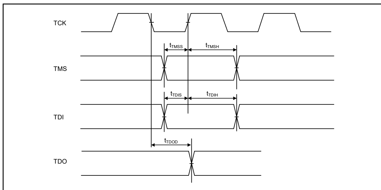
図 48.86 JTAG 入出力タイミング
