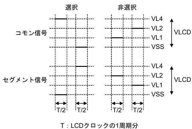
(d) 1/3バイアス法 (B波形)
