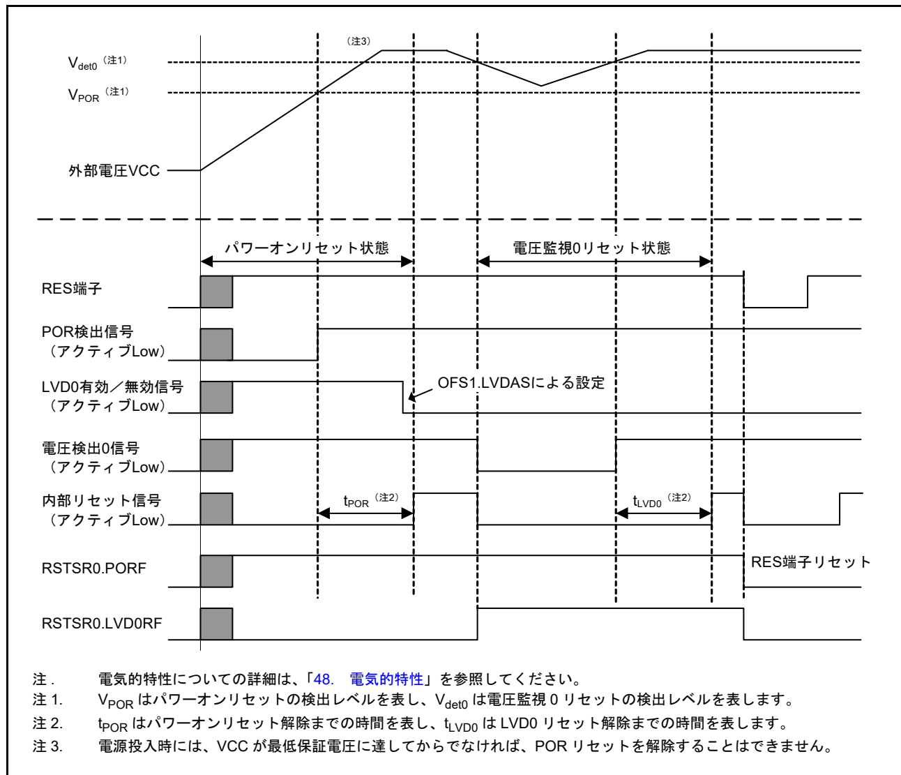
図 7.4 電圧監視 0 リセットの動作例
