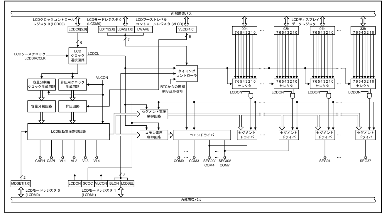
図 45.1 SLCDC のブロック図
