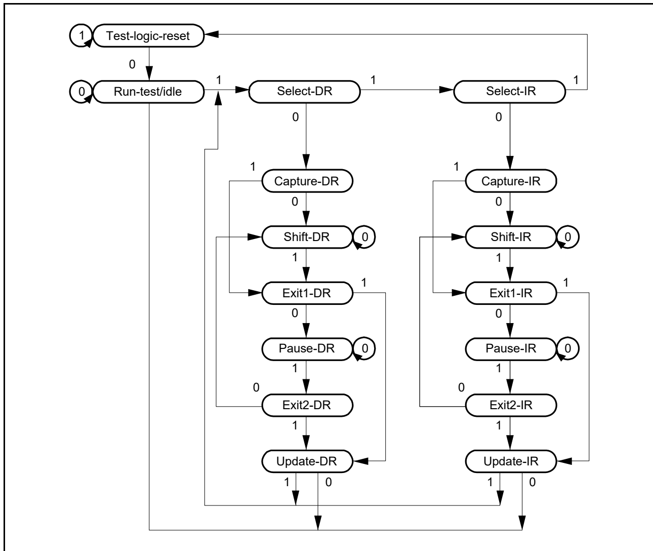
図 34.2 TAP コントローラの状態遷移図
