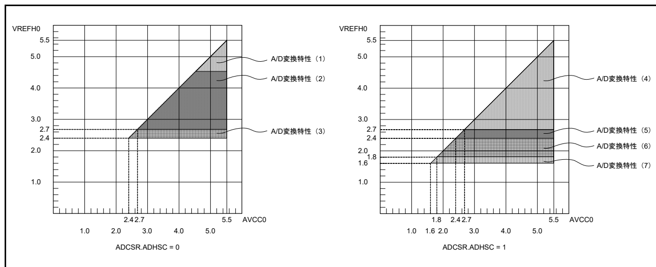
図 48.68 AVCC0 ~ VREFH0 電圧範囲
