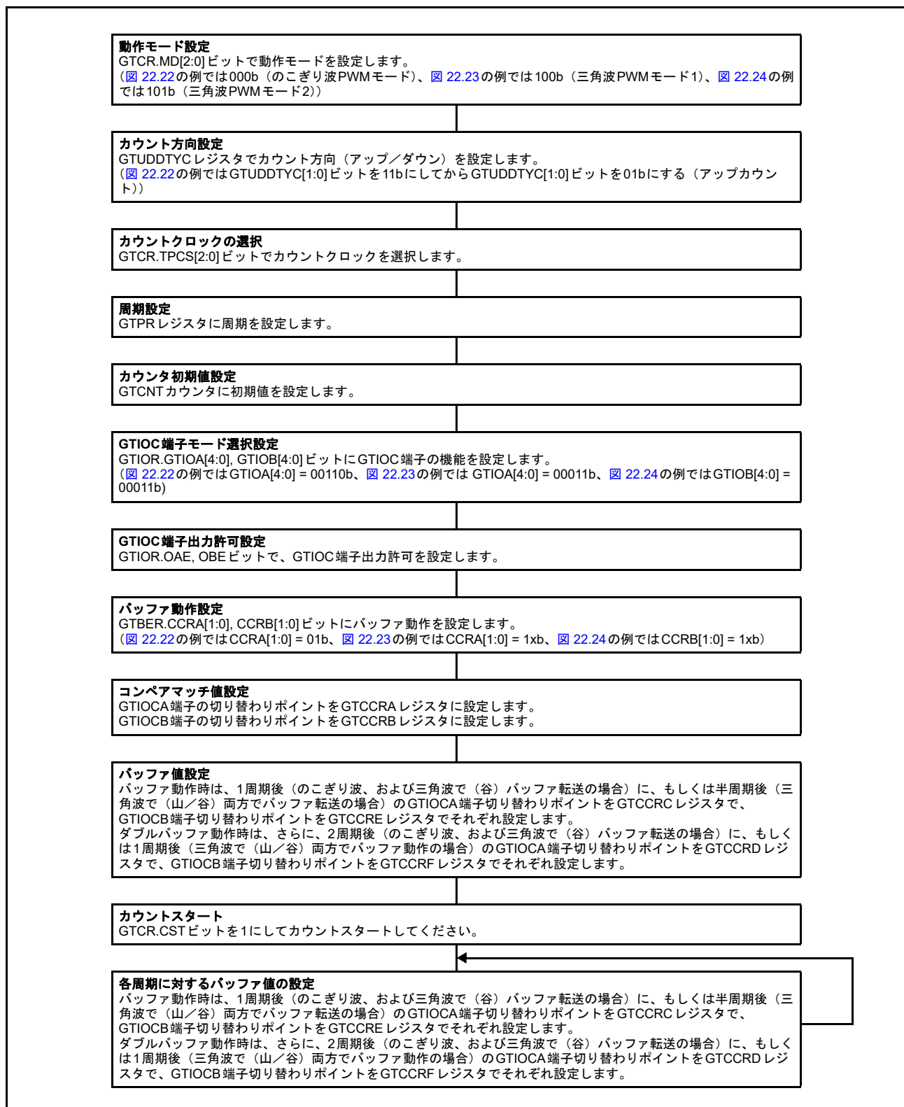
図 22.25 GTCRA、GTCCRB レジスタのバッファ動作の設定例 (アウトプットコンペア時)
