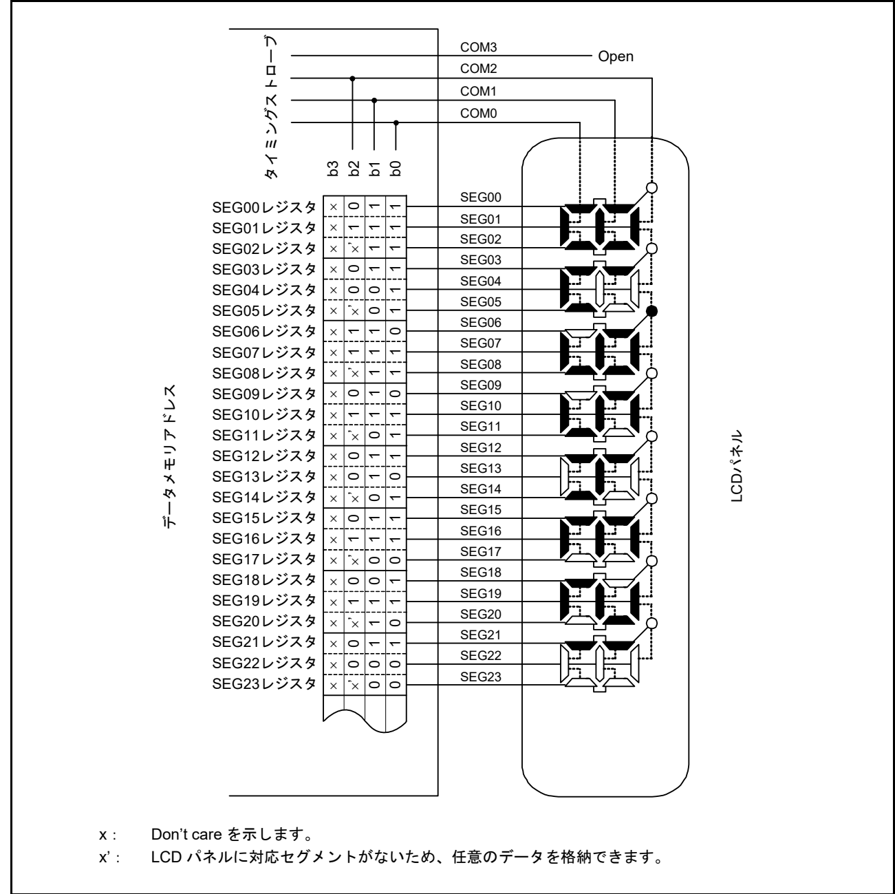
図 45.25 3 時分割 LCD パネルの接続例
