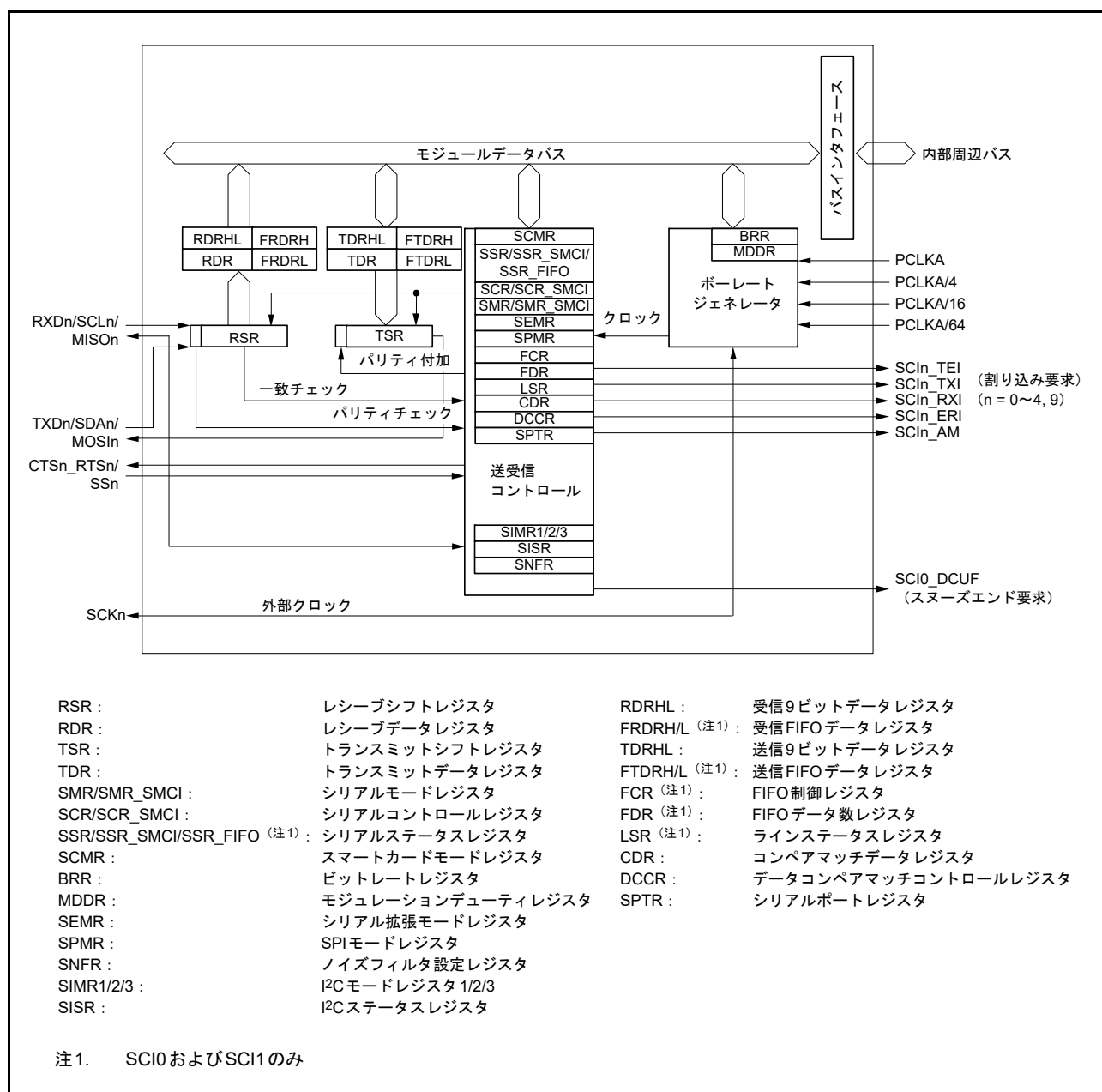
図 28.1 SCIのブロック図
