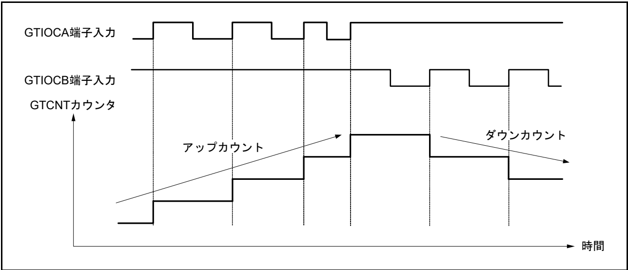
図 22.72 位相計数モード3 動作例 (B)
