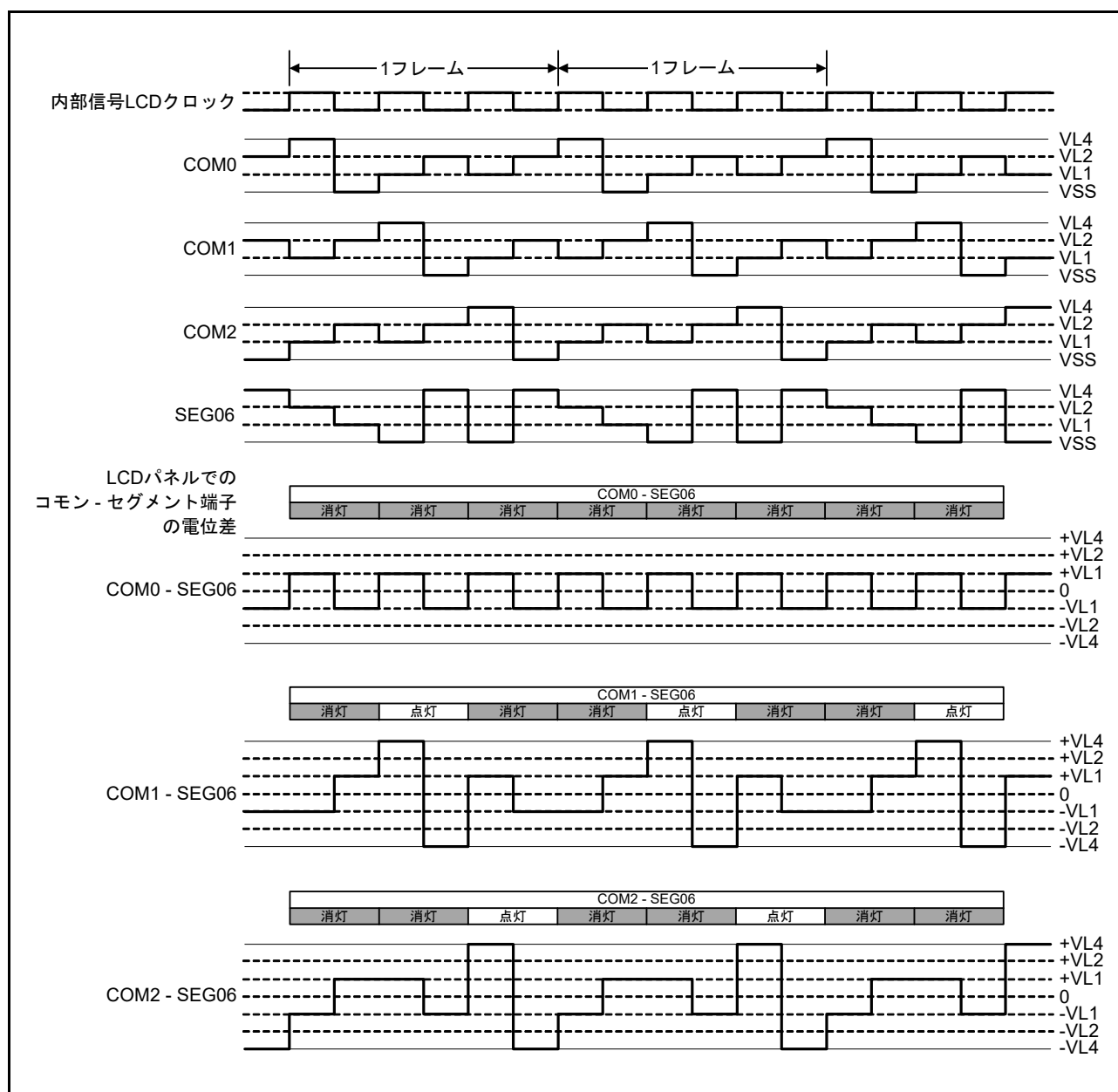
図 45.27 1/3 バイアス法を用いた SEG06 と各コモン信号との間の 3 時分割 LCD 駆動波形例
