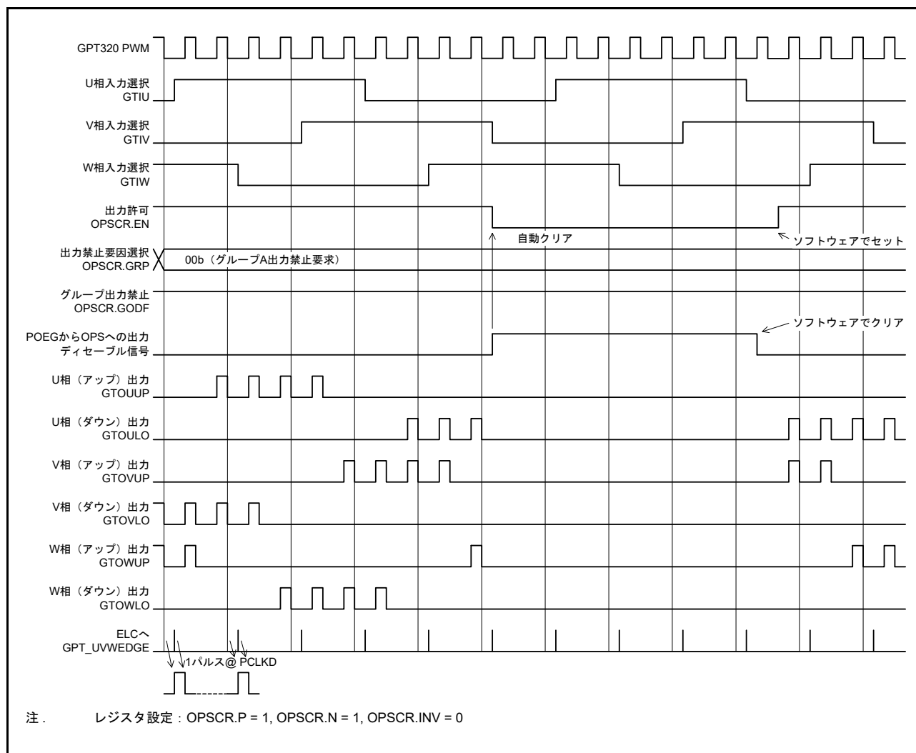
図 22.80 グループ出力禁止制御動作例
