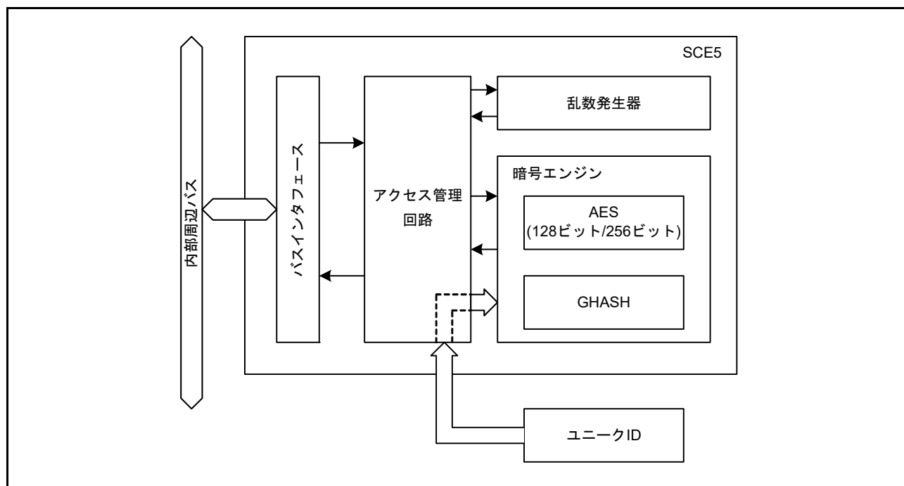
図 46.1 SCE5 ブロック図
