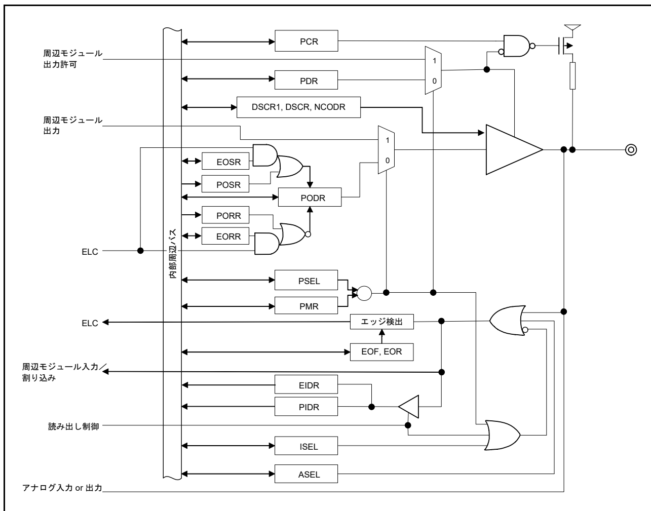
図 19.1 I/Oポートレジスタの接続図
