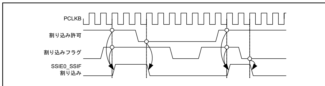
図 33.55 割り込み要因共通のタイミング図 (SSIE0_SSIF)
