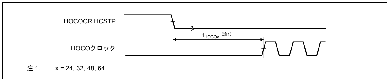
図 48.27 HOCO クロック発振開始タイミング (HOCOCR.HCSTP ビット設定による開始)
