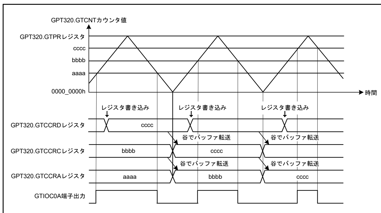
図 22.23 GTCRA、GTCCRB レジスタのダブルバッファ動作例（アウトプットコンペア、三角波、谷でバッファ動作、GTCCRA レジスタのコンペアマッチでトグル出力、周期の終わりで出力保持の場合）
