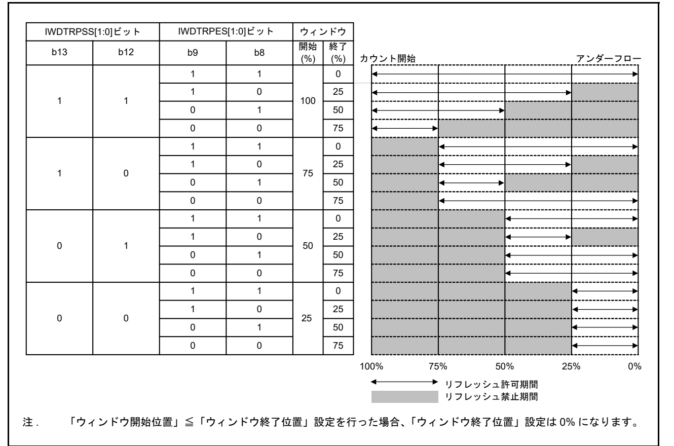
図 26.2 IWDTRPSS[1:0] および IWDTRPES[1:0] ビットとリフレッシュ許可期間
