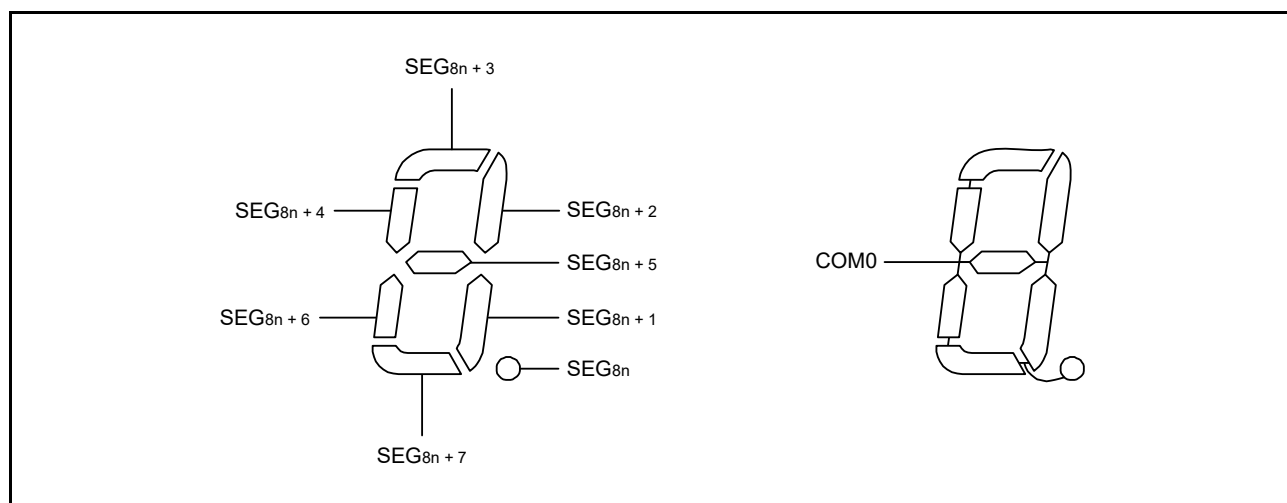
図 45.18 スタティク LCD 表示パターンと電極接続
