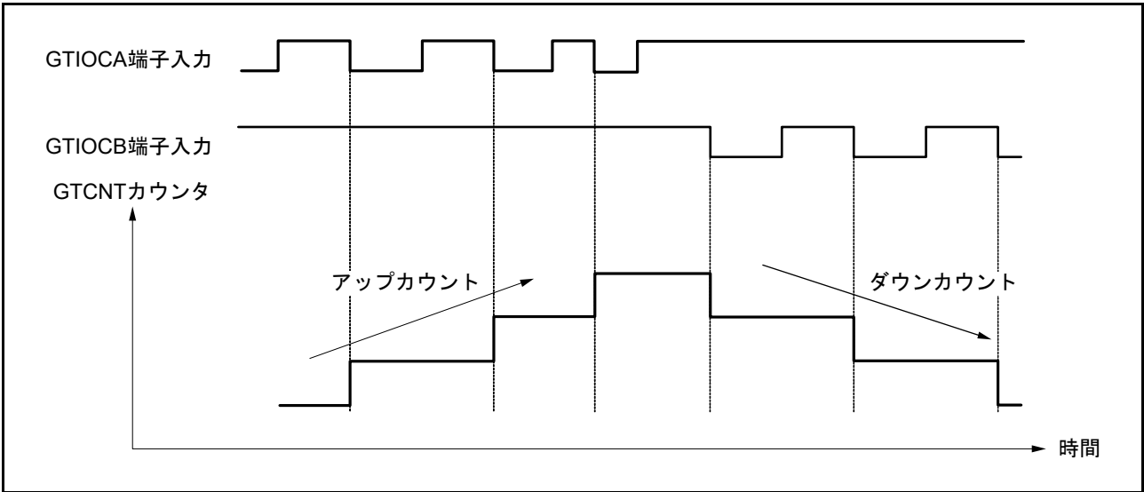
図 22.71 位相計数モード3 動作例（A）
