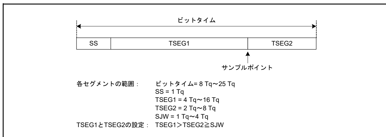
図 30.12 ビットタイミング
