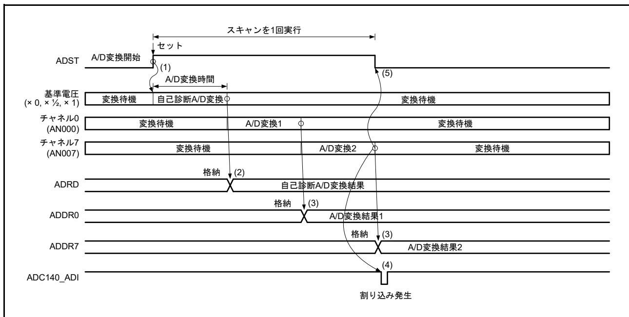
図 35.7 シングルスキャンモードの基本動作例 (AN000、AN007 選択 + 自己診断)
