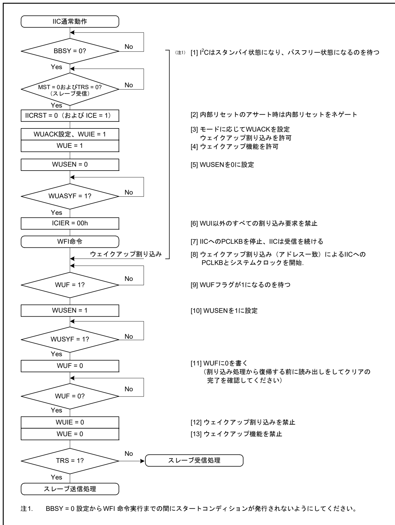
図 29.30 ノーマルウェイクアップモード1の動作例（スレープアドレス一致時のウェイクアップ割り込みによるウェイクアップの場合）
