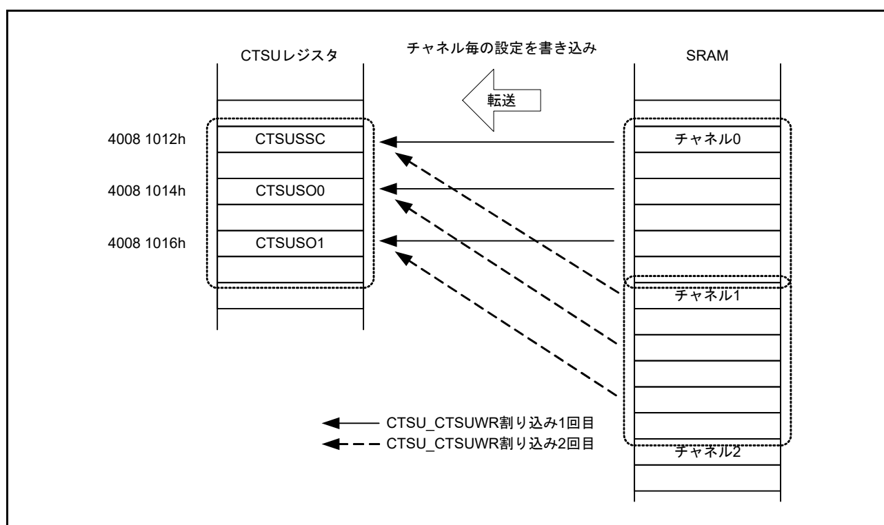
図 41.19 CTSUS_CTSUWR 割り込みを用いた DTC 転送動作例
