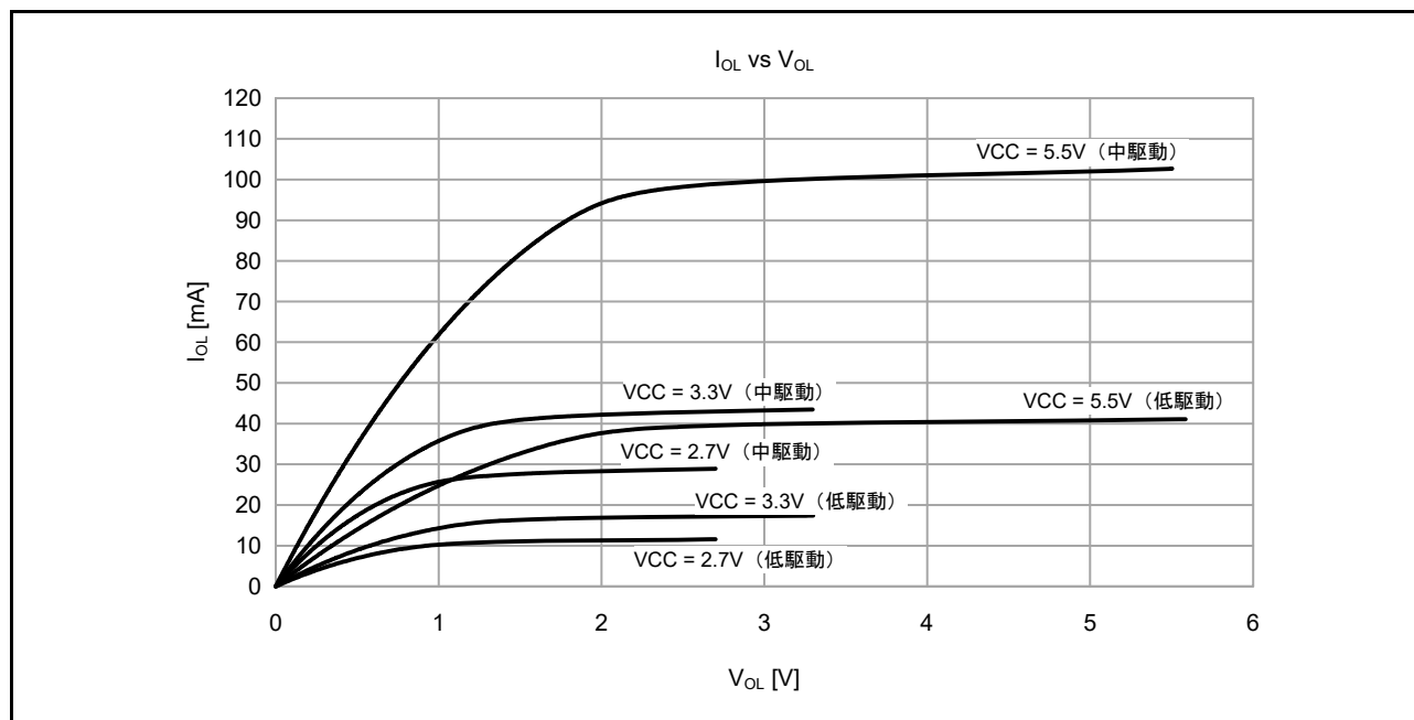
図 48.16 T_a = 25^\circ\text{C} での V_{OH}/V_{OL} および I_{OH}/I_{OL} 電圧特性
