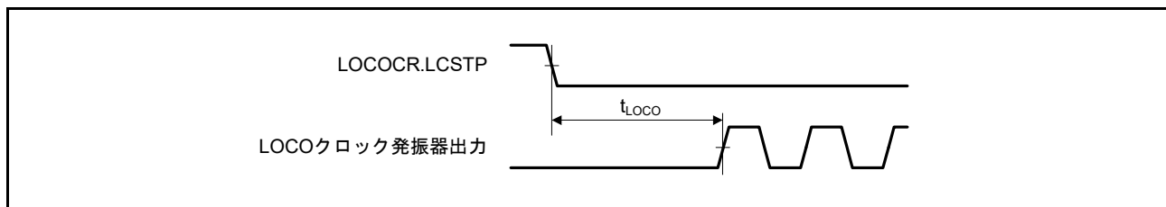
図 48.26 LOCO クロック発振開始タイミング
