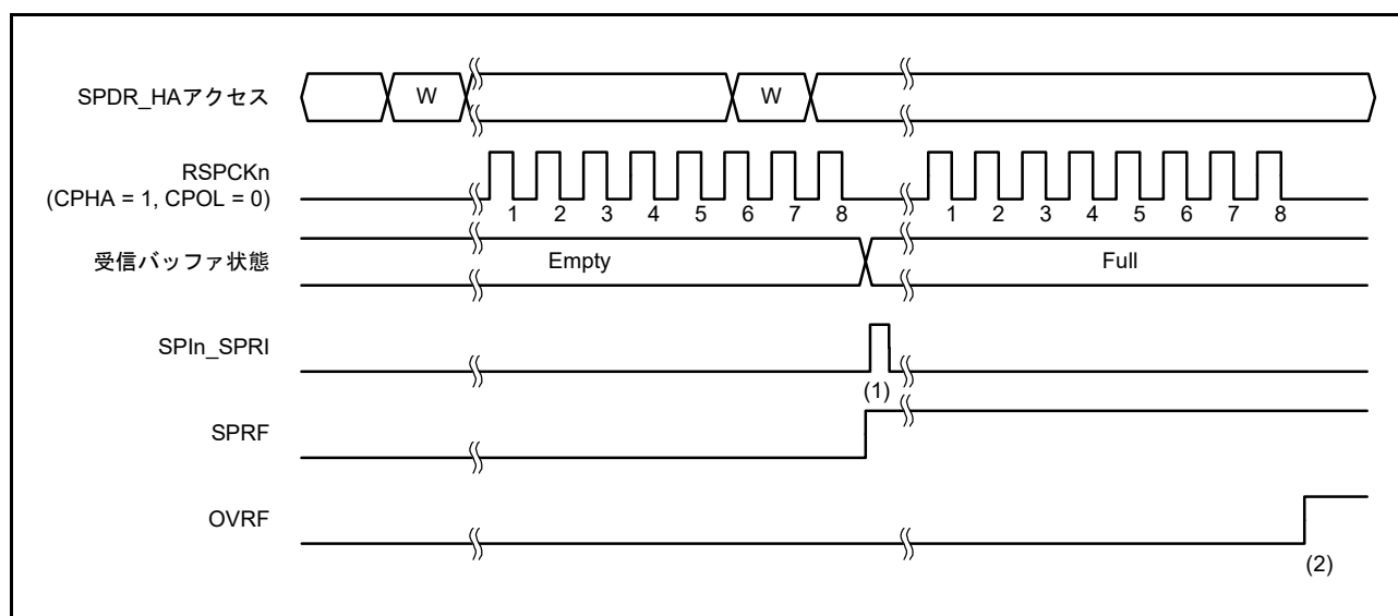
図 31.24 SPCR.TXMD = 0 の動作例
