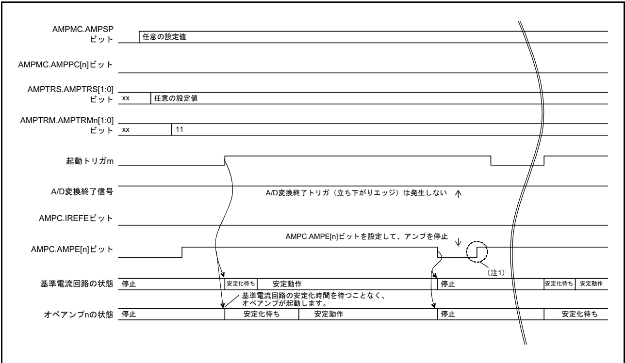
図 38.6 オペアンプの制御動作（起動および A/D トリガモード（2）） （基準電流回路およびオペアンプを起動トリガによって起動し、AMP レジスタの設定によって基準電流回路およびオペアンプを停止する場合）
