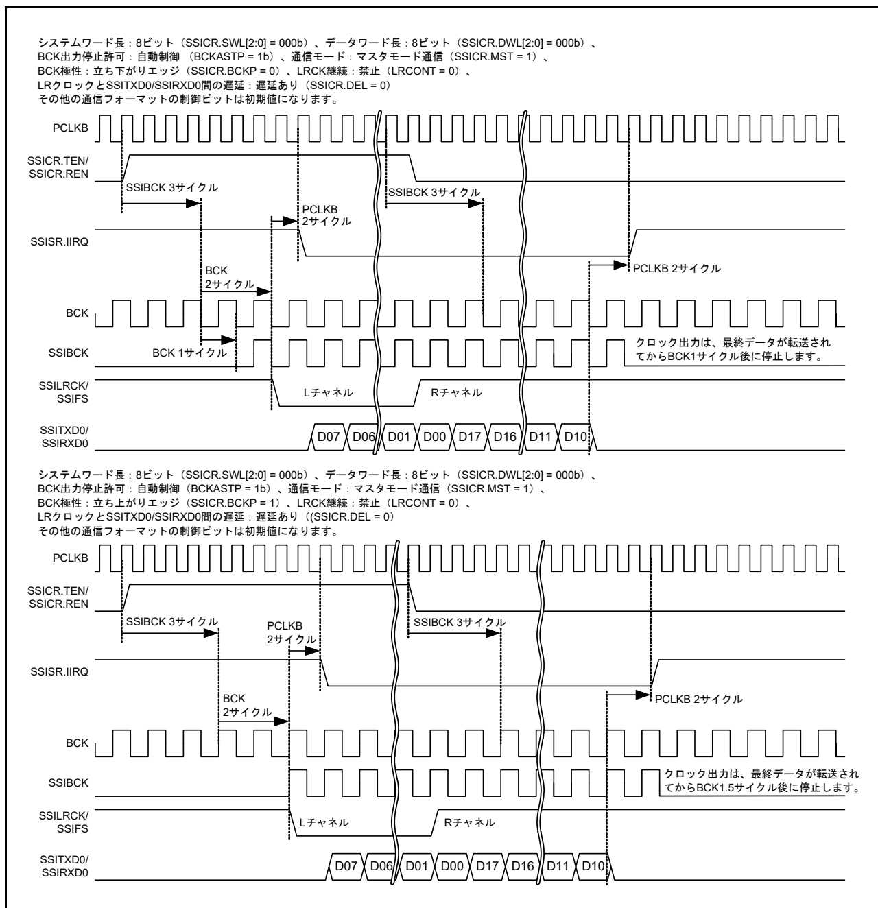
図 33.33 BCKASTP ビット通信動作の動作例 (BCKASTP = 1 の場合)
