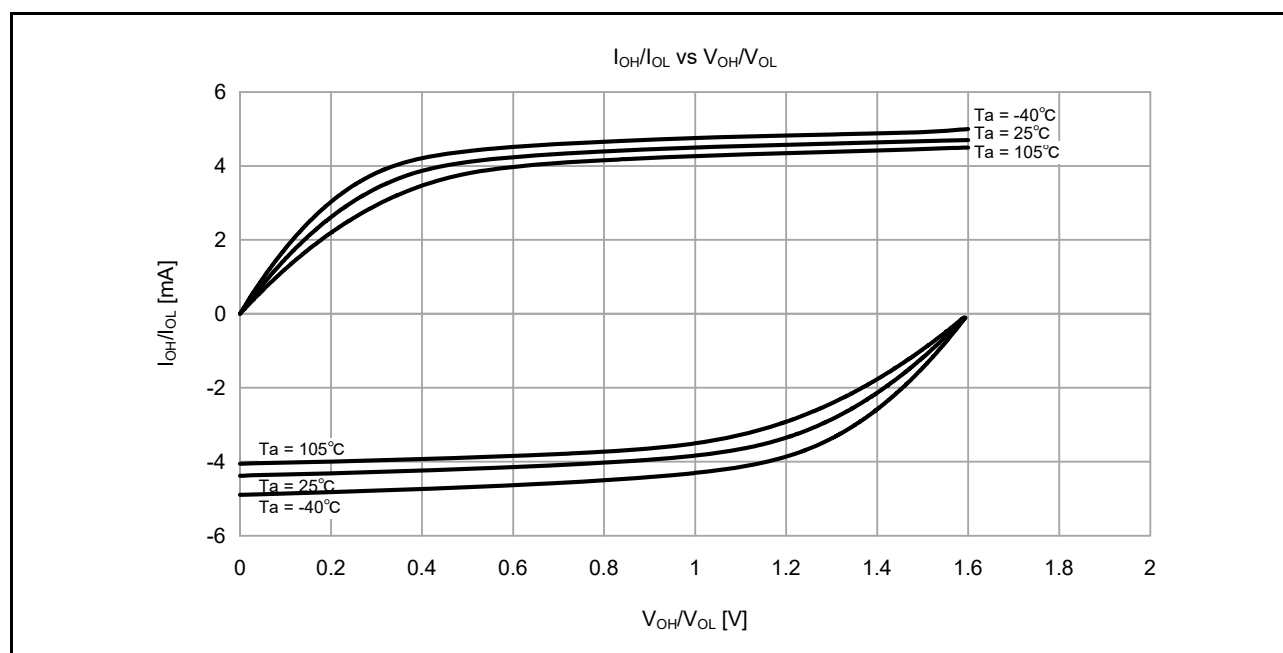
図 48.8 中駆動出力選択時の V_{CC} = 1.6\text{V} での V_{OH}/V_{OL} および I_{OH}/I_{OL} 温度特性 (参考データ)
