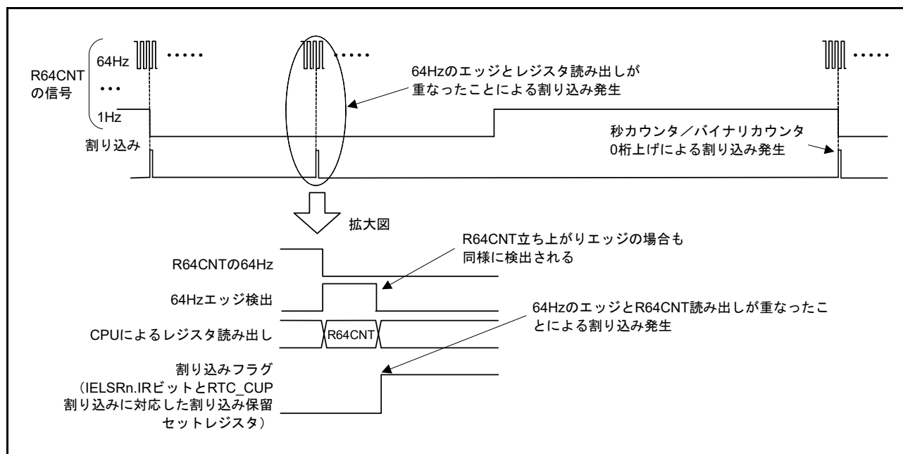
図 24.12 桁上げ割り込み (RTC_CUP) のタイミング
