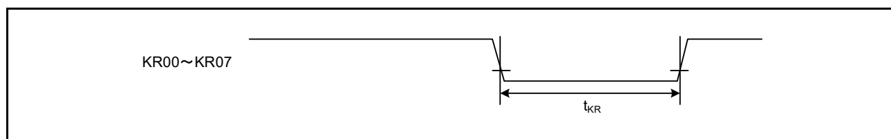
図 48.43 キー割り込み入力タイミング
