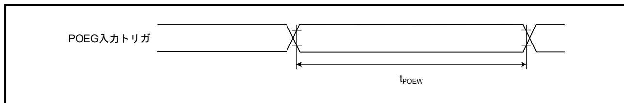
図 48.39 POEG 入力トリガタイミング
