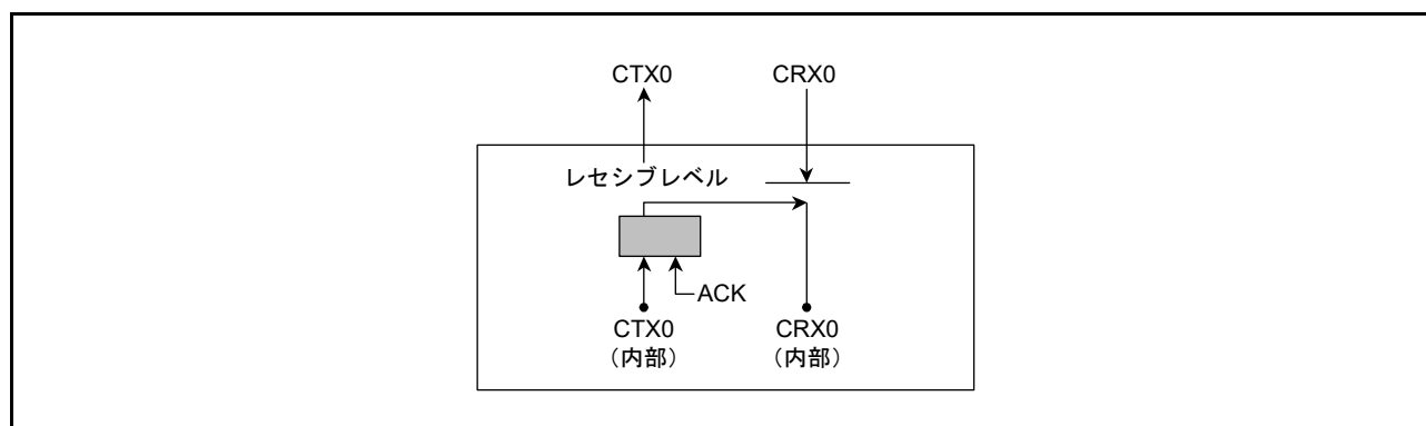
図 30.8 セルフテストモード 1 選択時の接続
