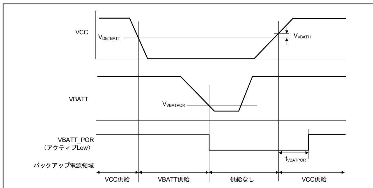
図 48.79 VBATT_POR リセットタイミング
