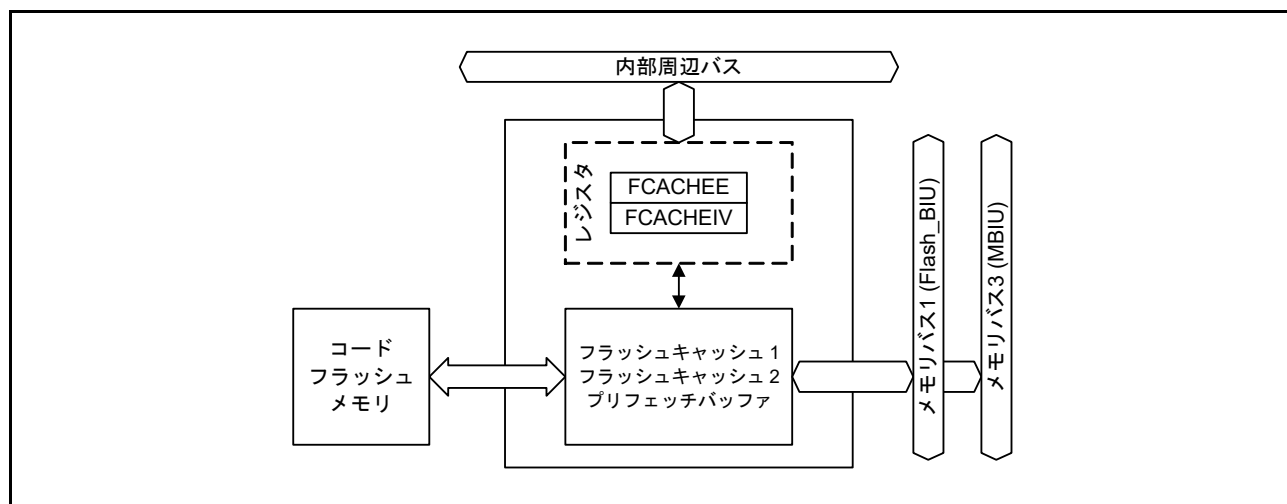
図 44.4 FCACHE のブロック図
