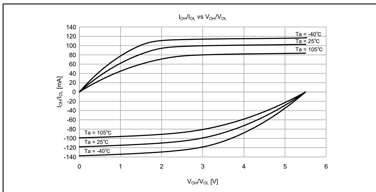
図 48.11 中駆動出力選択時の V_{CC} = 5.5\text{V} での V_{OH}/V_{OL} および I_{OH}/I_{OL} 温度特性 (参考データ)
