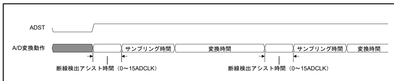
図 35.26 断線検出アシスト機能を使用した場合の A/D 変換動作図
