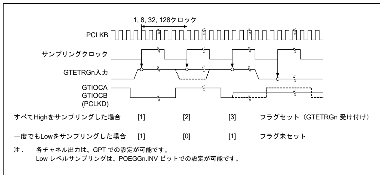
図 21.2 デジタルフィルタの動作例
