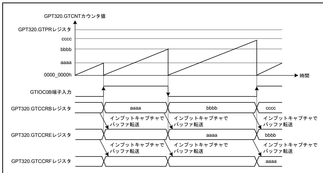
図 22.27 GTCCRA、GTCCRB レジスタのダブルバッファ動作例 (GTIOC0B 端子入力の両エッジでインプットキャプチャ、のこぎり波でアップカウント、GTIOC0B 端子入力の両エッジで GTCNT カウンタクリアの場合)
