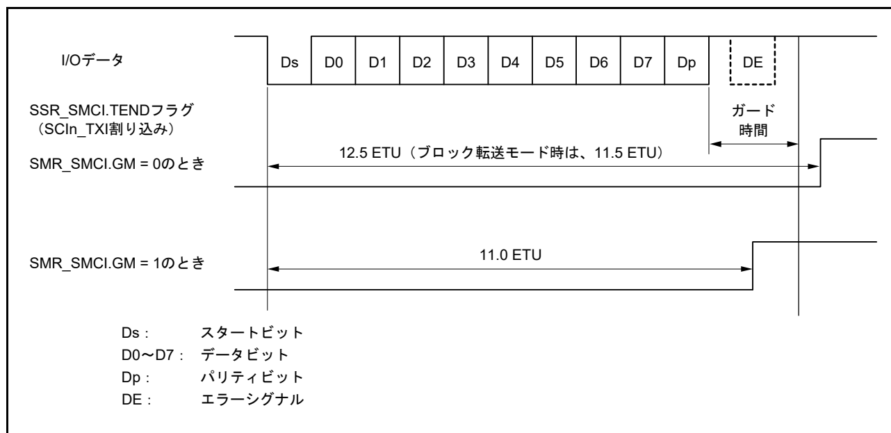
図 28.53 送信中の SSR.TEND フラグの発生タイミング
