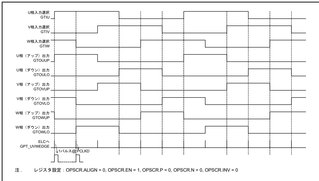
図 22.78 6 相レベル出力動作例
