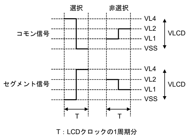
(c) 1/3バイアス法 (A波形)
