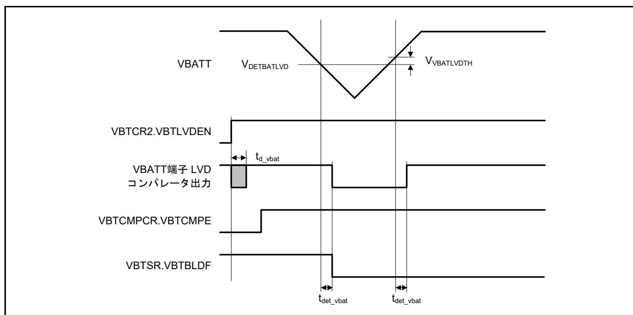
図 48.80 VBATT 端子電圧検出回路タイミング
