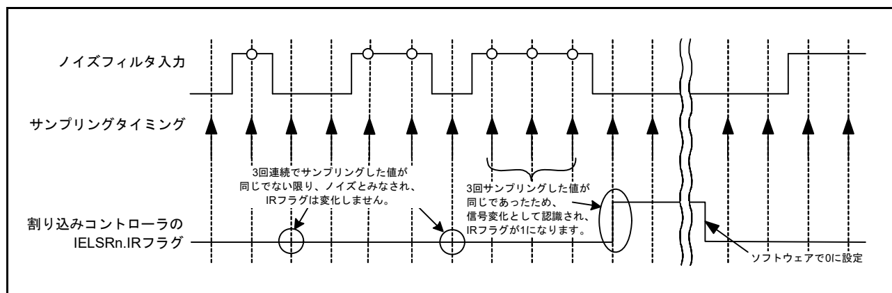
図 39.6 ノイズフィルタおよび割り込みの動作例
