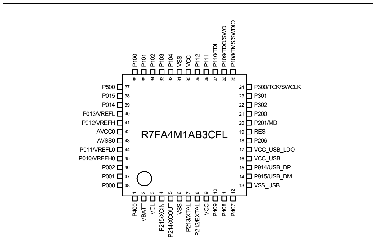
図 1.7 48-pin LQFP のピン配置図 (上面図)
