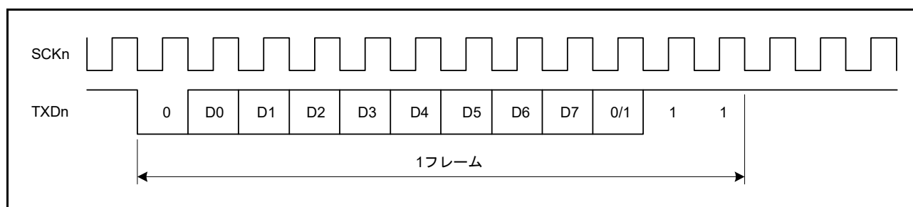
図 28.4 出力クロックと送信データの位相関係 (調歩同期式モード: SCMR.CHR1 = 1、SEMR.CHR = 0、PE = 1、MP = 0、STOP = 1)
