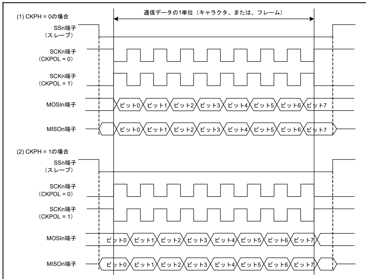
図 28.70 簡易 SPI モードにおけるクロックと送受信データの関係
