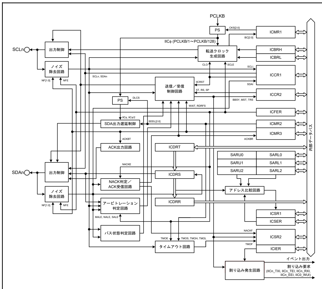
図 29.1 IIC のブロック図
