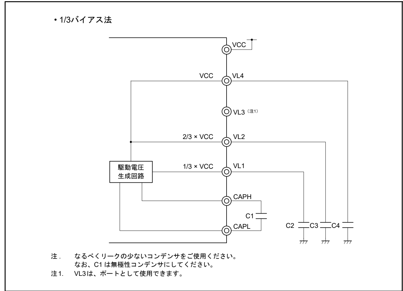
図 45.12 LCD 駆動電源の接続例（容量分割方式）
