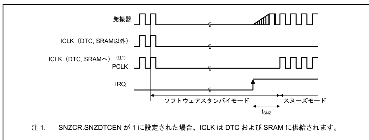
図 48.35 ソフトウェアスタンバイモードからスヌーズモードへの復帰タイミング
