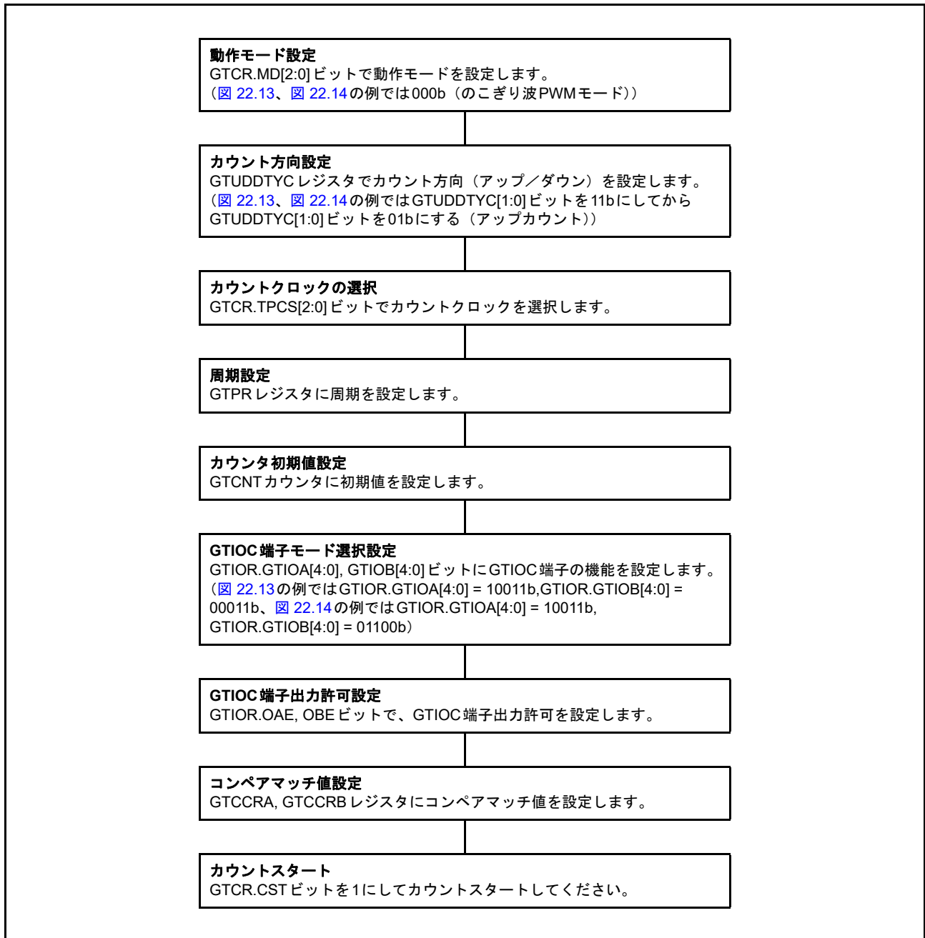
図 22.15 トグル出力動作の設定例
