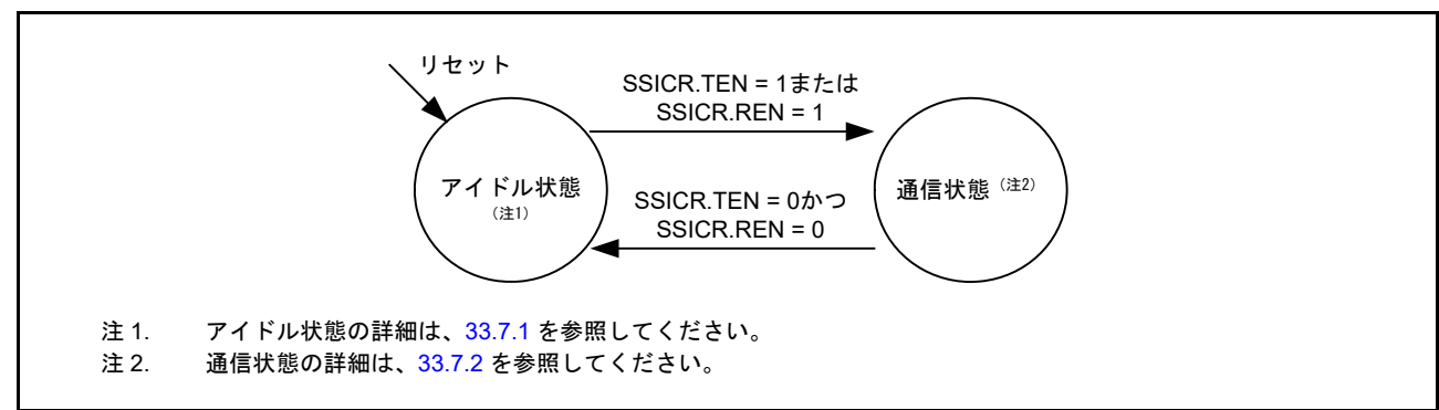
図 33.39 SSIE の状態遷移
