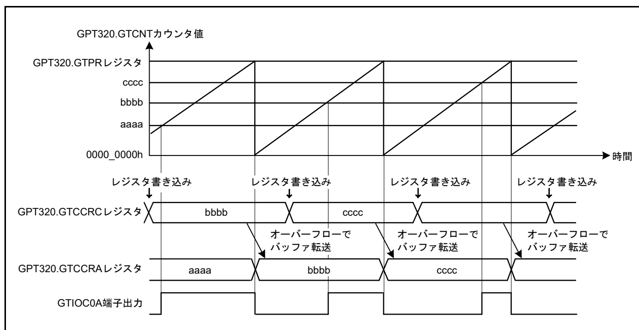
図 22.22 GTCRA、GTCCRB レジスタのバッファ動作例（アウトプットコンペア、アップカウント時ののこぎり波、GTCCRA レジスタのコンペアマッチで High 出力、周期の終わりで Low 出力の場合）
