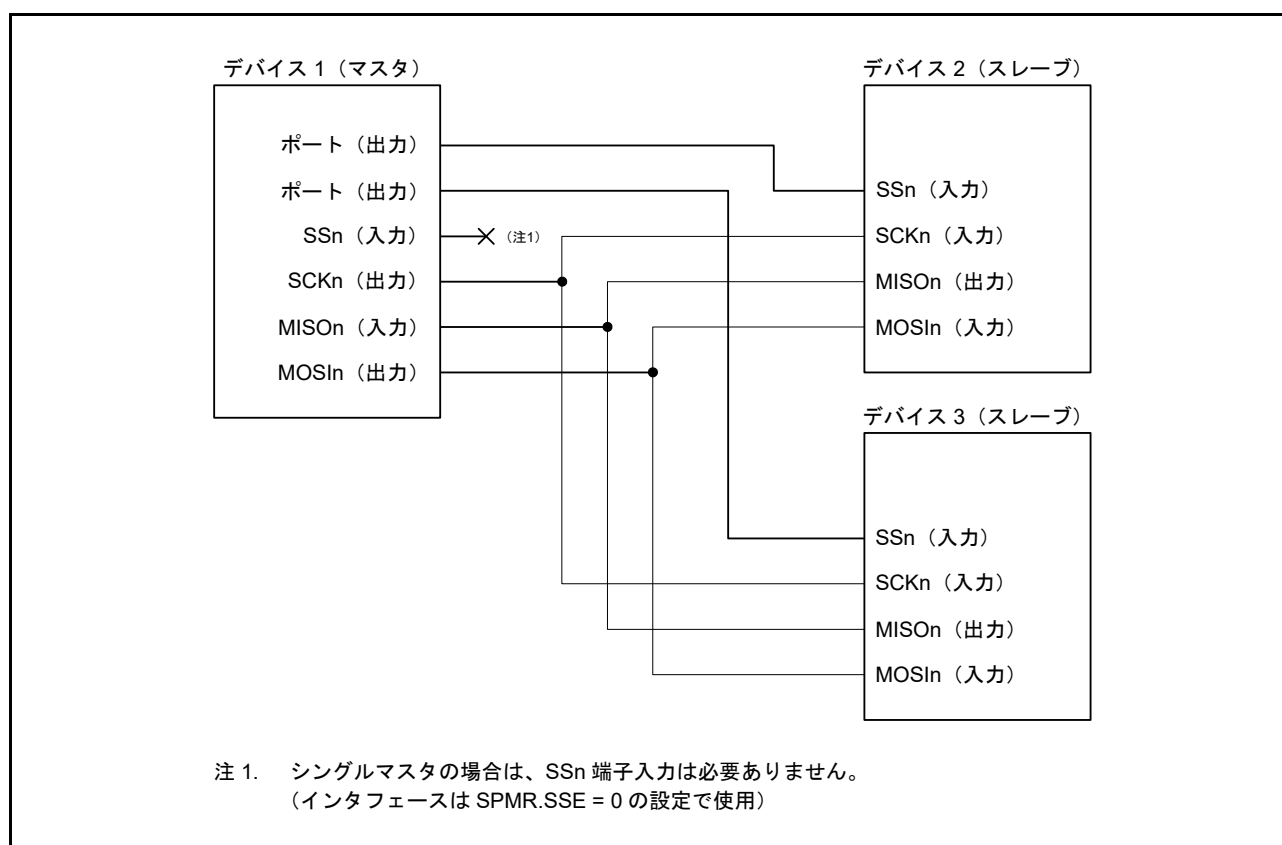
図 28.69 簡易 SPI モードでの接続例 (シングルマスタ時、SPMR.SSE ビット = 0)
