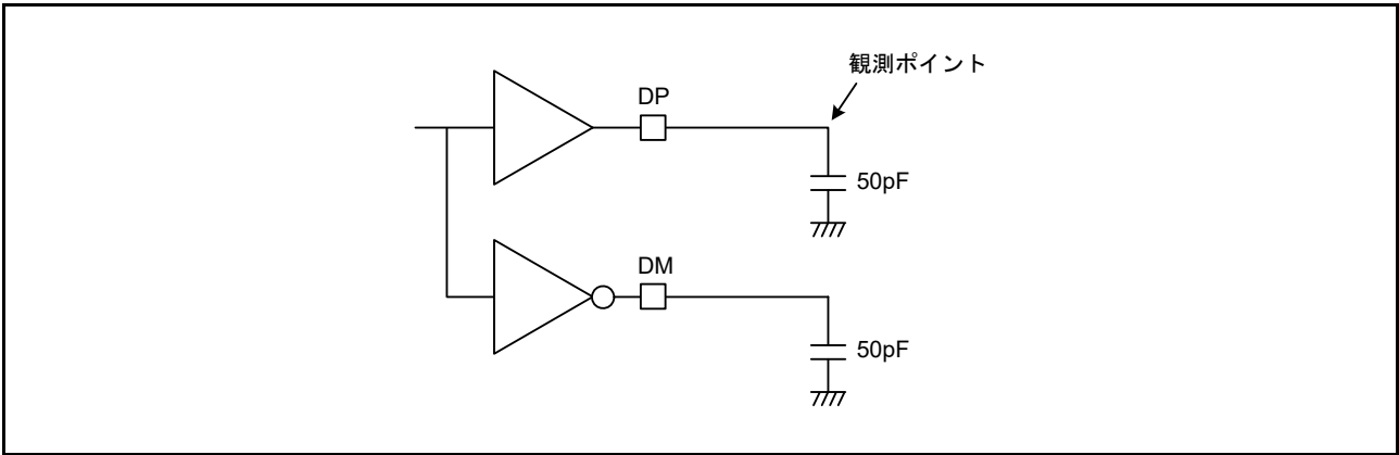
図 48.66 フルスピード（FS）接続の測定回路
