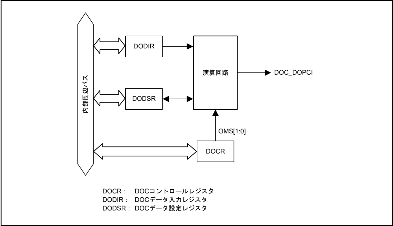
図 42.1 DOC ブロック図
