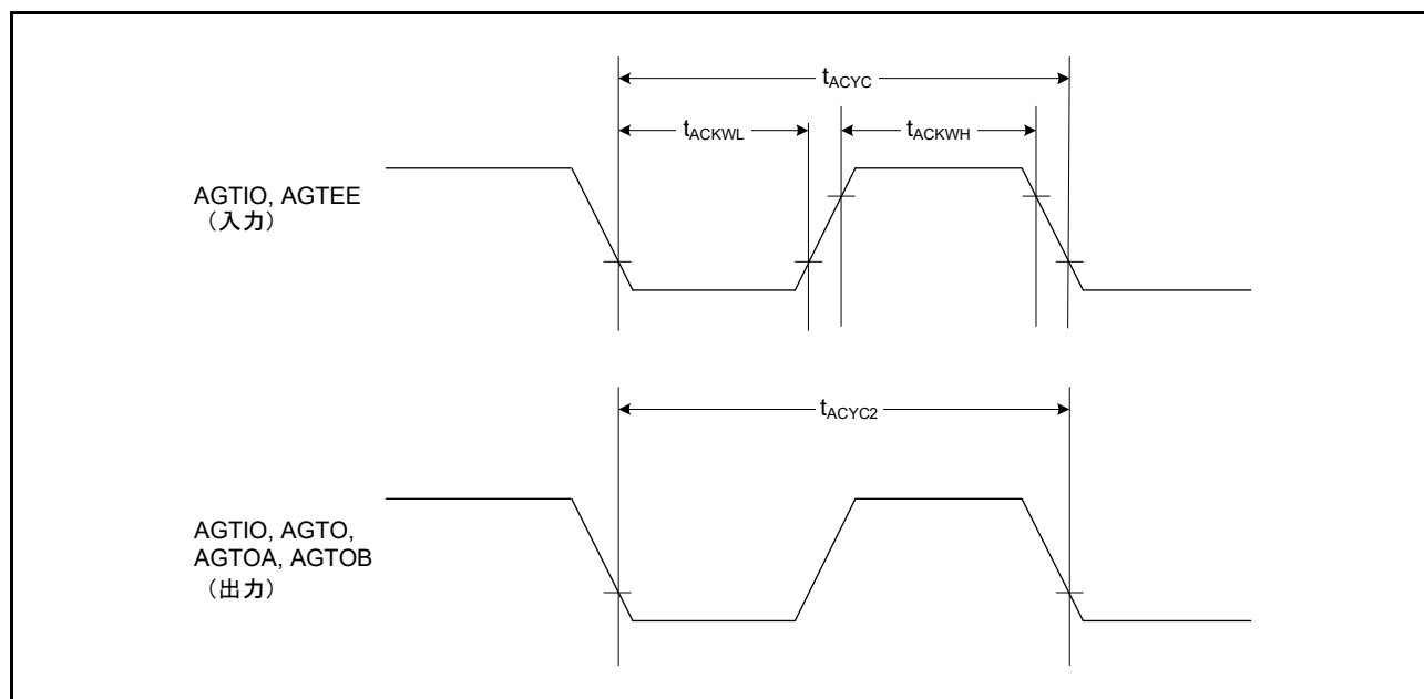
図 48.41 AGT 入出力タイミング
