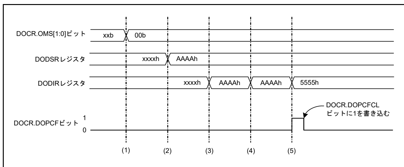
図 42.2 データ比較モードの動作例
