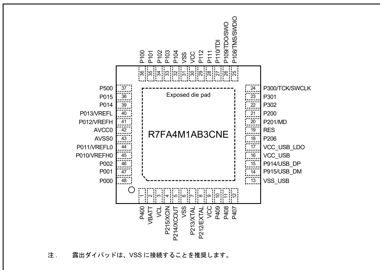
図 1.8 48-pin QFN のピン配置図（上面図）
