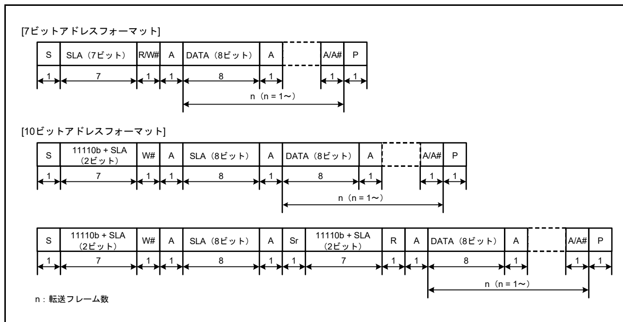
図 29.3 I 2 C バスフォーマット
