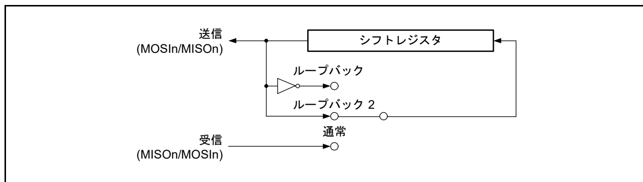
図 31.42 ループバックモード時のシフトレジスタ入出力経路の構成 (マスタモード)
