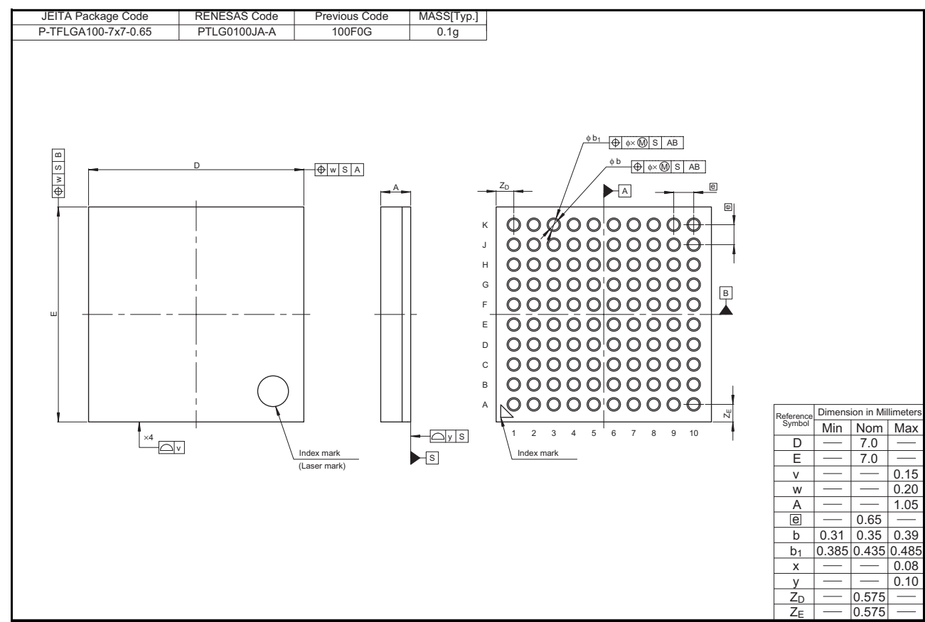
図 2.1 100-pin LGA
