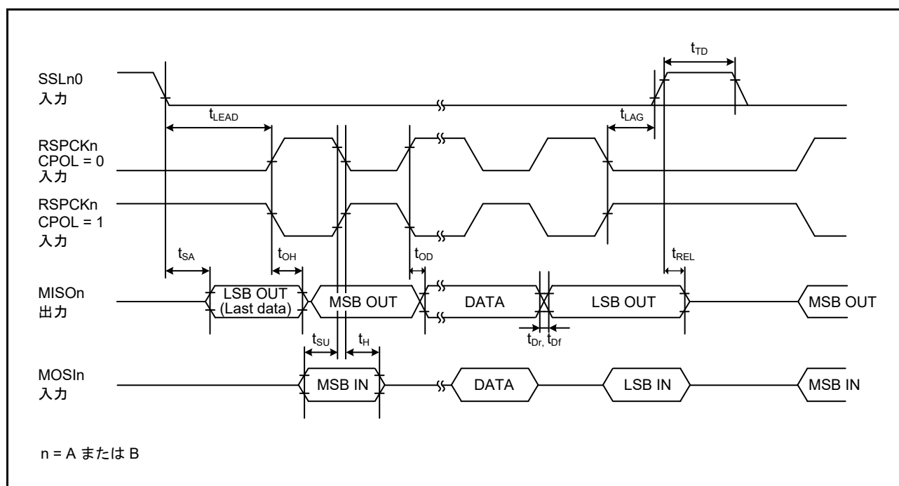
図 48.58 SPI タイミング (スレーブ、CPHA = 1)
