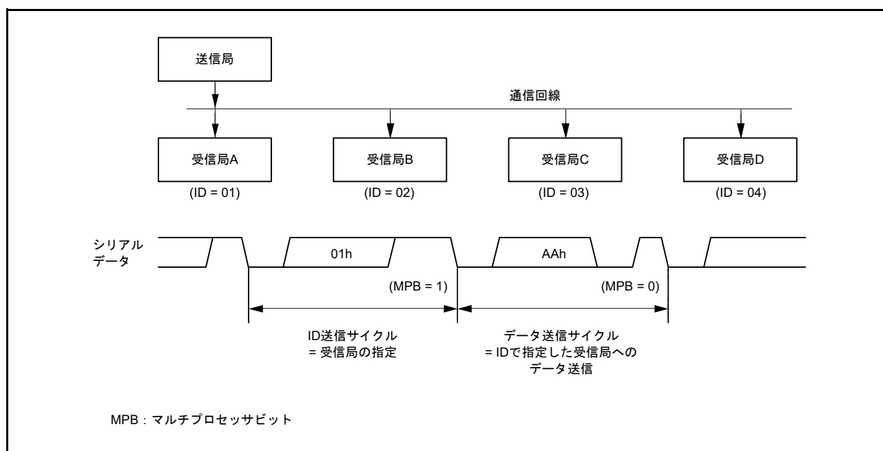
図 28.22 マルチプロセッサフォーマットを使用した通信例（データ AAh を受信局 A に送信する場合）
