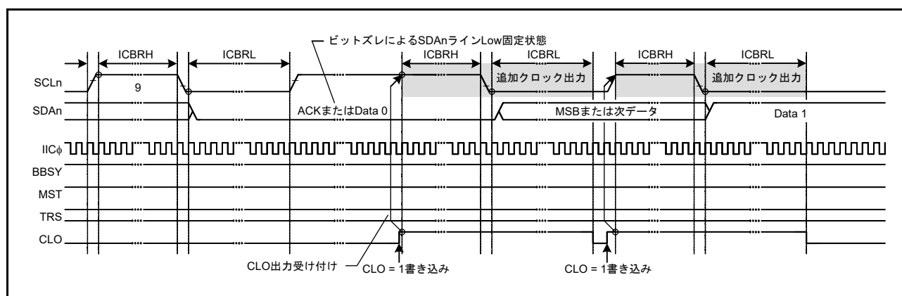
図 29.49 SCL クロック追加出力機能 (CLO ビット)
