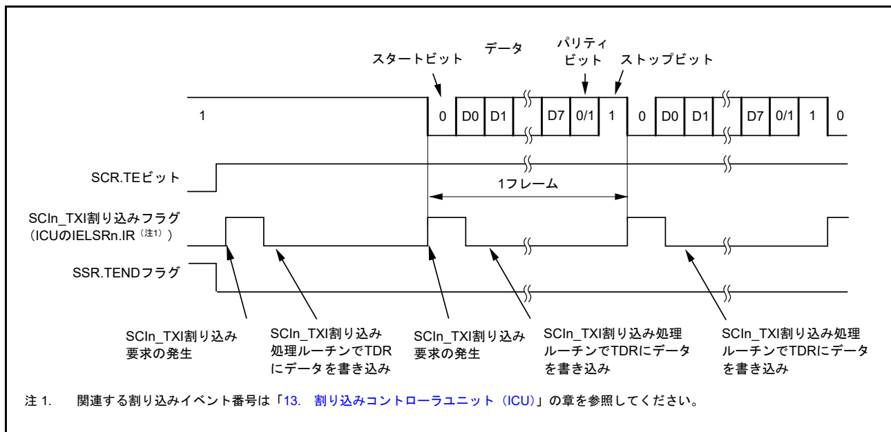
図 28.9 調歩同期式モードにおけるシリアル送信の動作例 (1) (8 ビットデータ/パリティあり/1 ストップビット/CTS 機能不使用/送信開始時)
