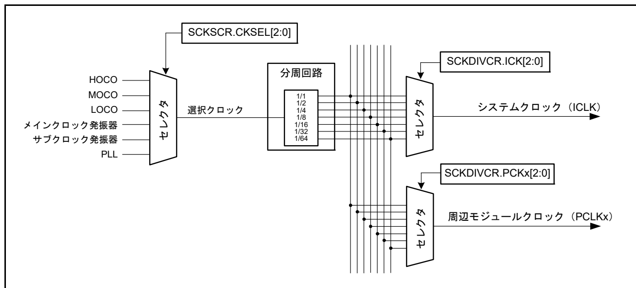
図 8.8 クロックソース選択ブロック図
