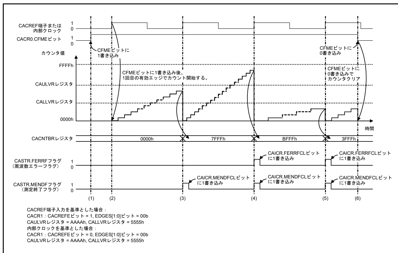
図 9.2 CAC の動作例
