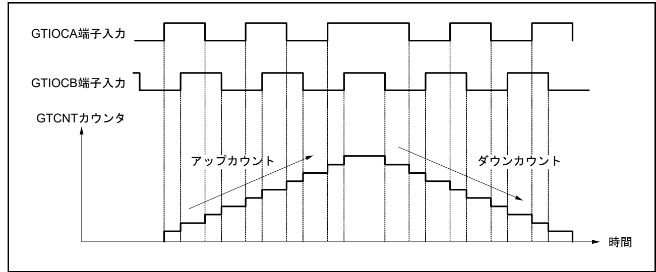
図 22.67 位相計数モード 1 動作例
