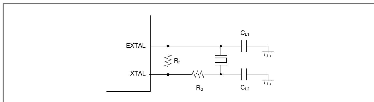
図 8.4 水晶振動子の接続例
