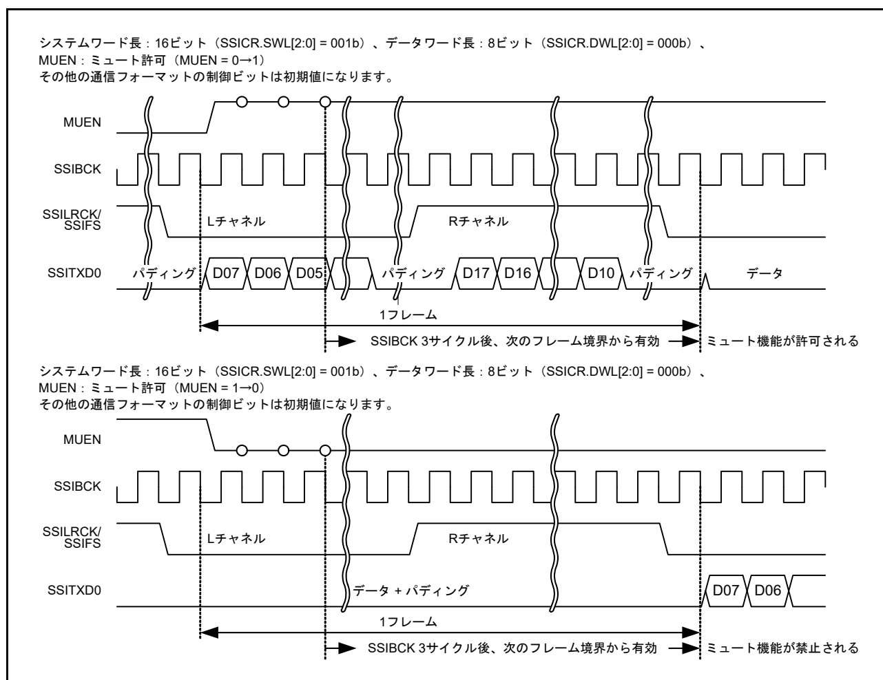
図 33.4 ミュート機能設定時の送信データ
