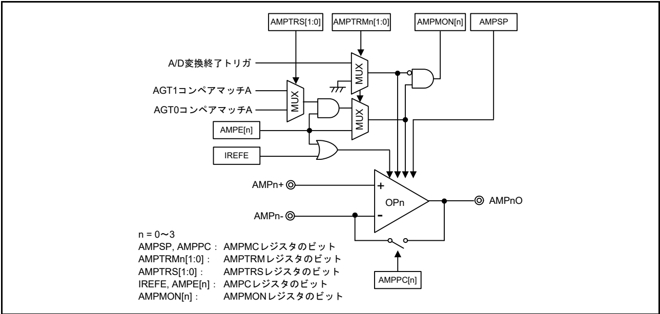
図 38.1 オペアンプのブロック図
