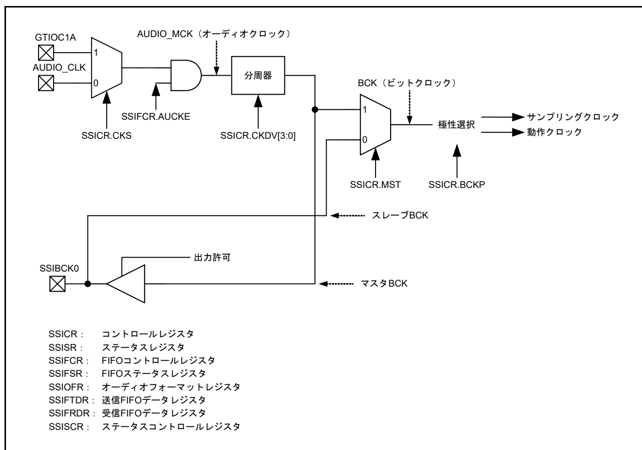
図 33.3 SSIE クロック構成
