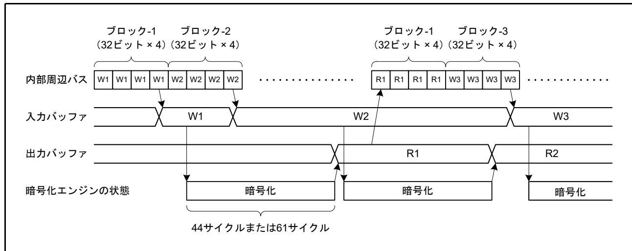
図 46.3 暗号化と復号タイミング (AES)
