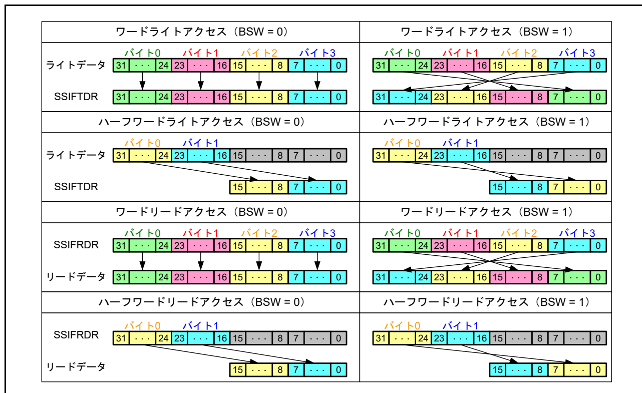
図 33.22 バイトスワップの動作例
