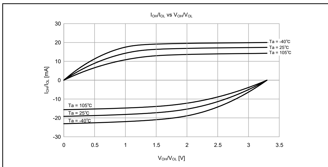
図 48.5 低駆動出力選択時の V_{CC} = 3.3\text{V} での V_{OH}/V_{OL} および I_{OH}/I_{OL} 温度特性 (参考データ)
