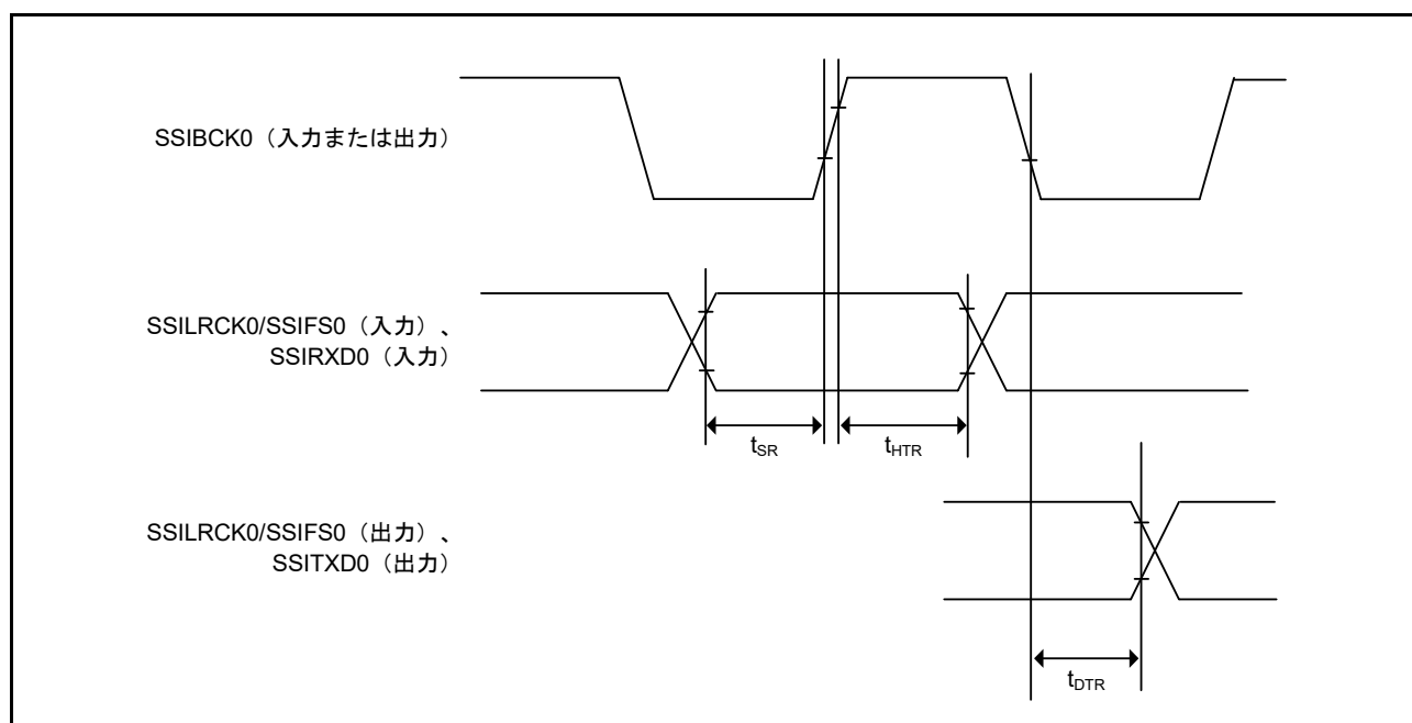
図 48.61 SSIE データ送受信タイミング (SSICR.BCKP = 0)
