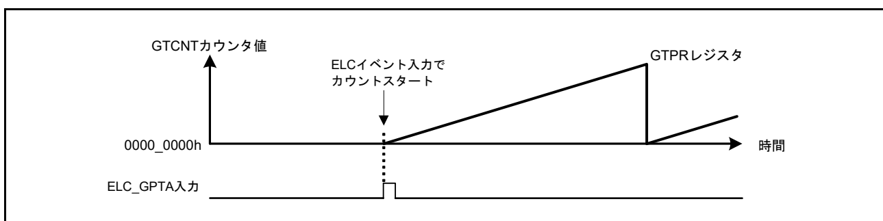
図 22.47 ハードウェア要因によるカウントスタート動作例 (ELC_GPTA イベントからの信号入力時のスタート)
