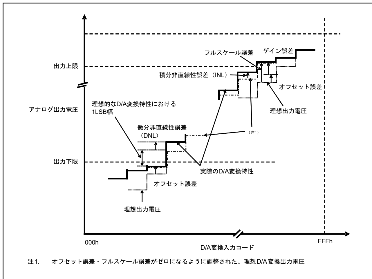
図 48.71 D/A コンバータ特性用語の解説図
