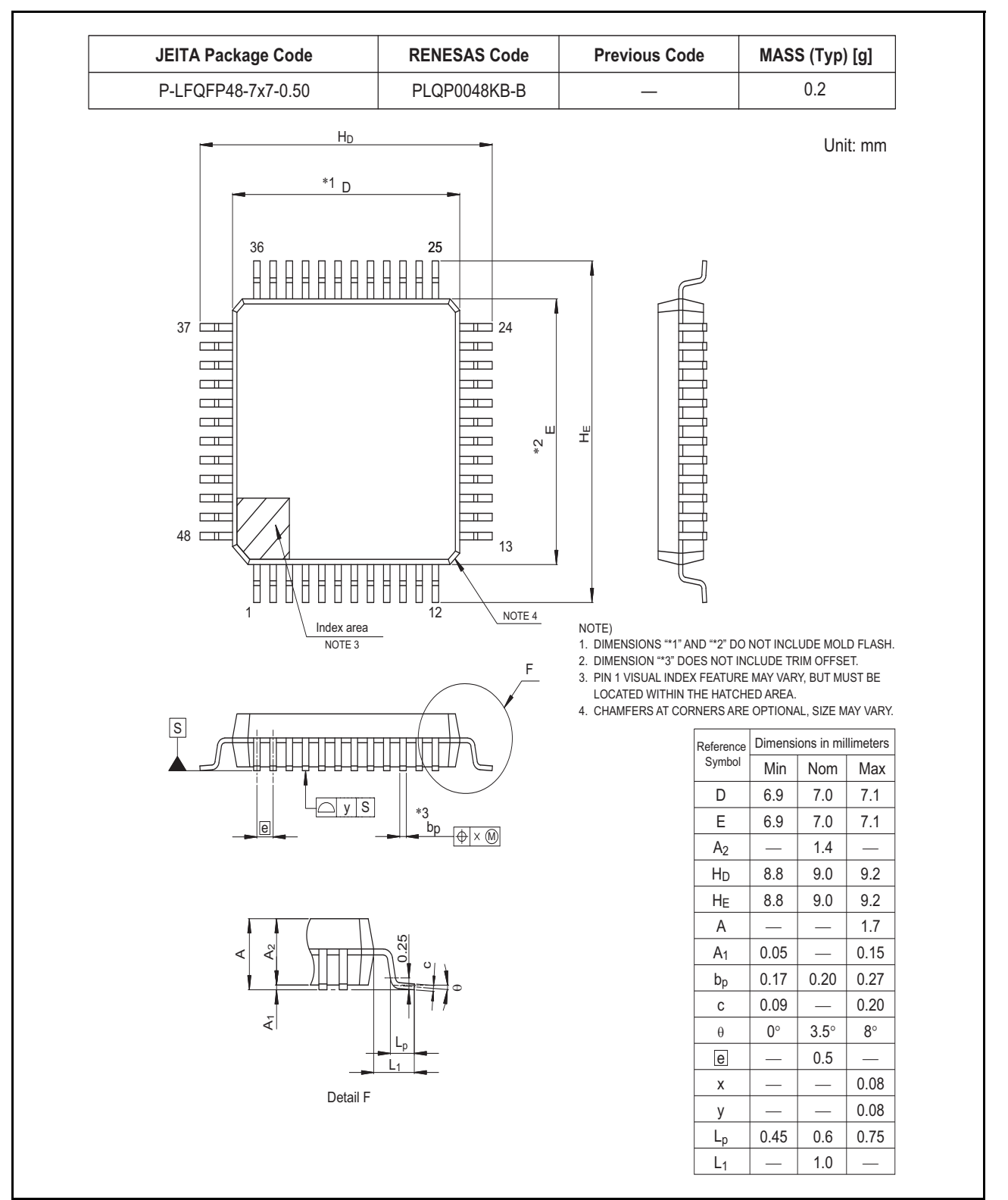
図 2.6 48-pin LQFP
