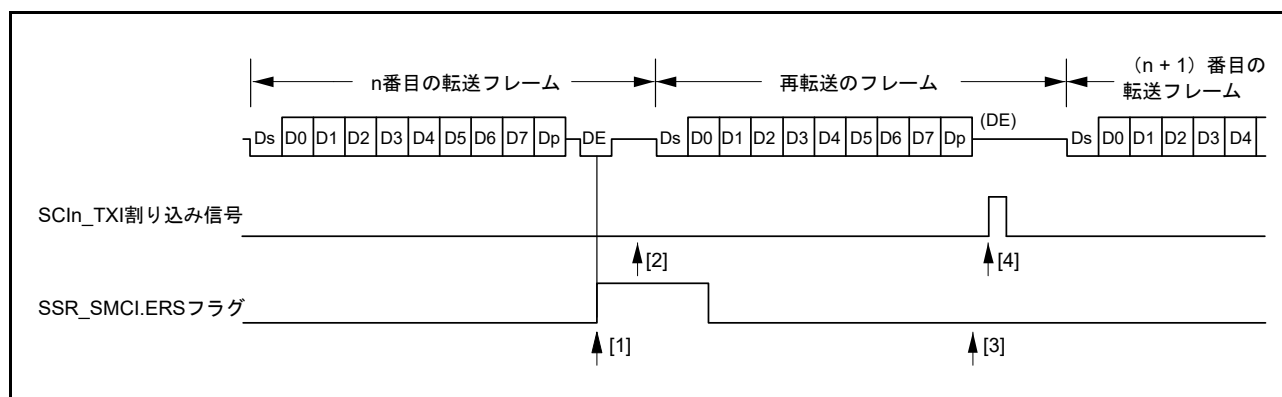
図 28.52 スマートカードインタフェース送信モードでのデータ再転送動作
