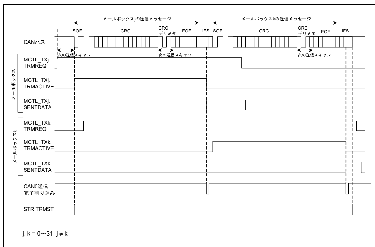
図 30.20 データフレーム送信時の動作例
