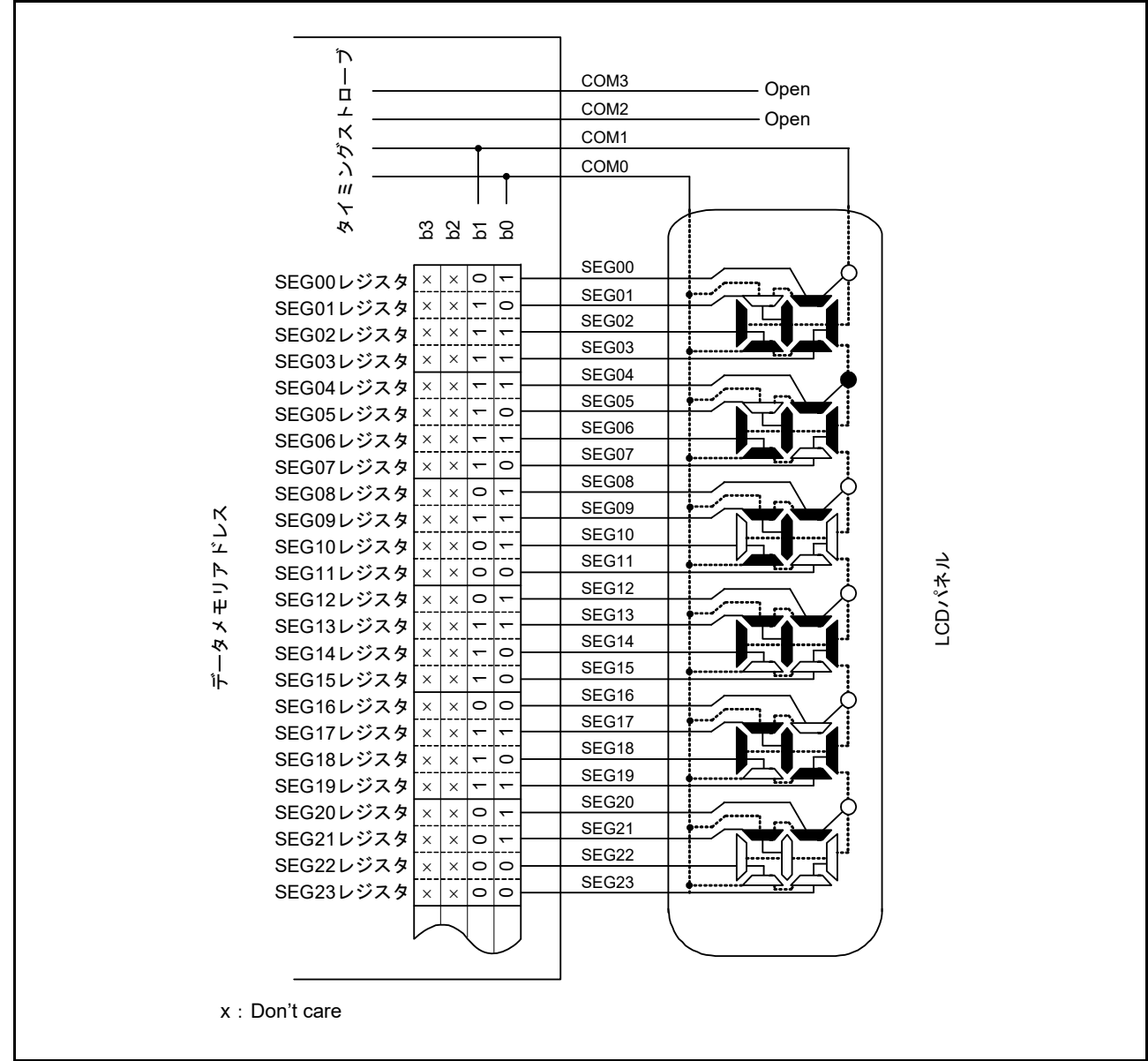
図 45.22 2 時分割 LCD パネルの接続例
