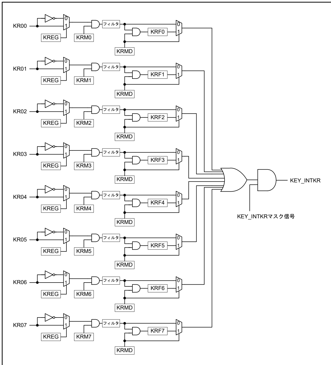
図 20.1 キー割り込み機能のブロック図
