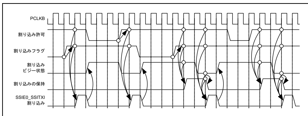
図 33.56 SSIE0_SSITXI 割り込みのタイミング図
