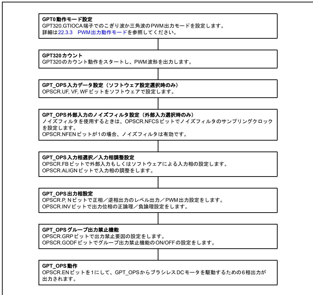
図 22.81 GPT_OPS スタート動作の設定例
