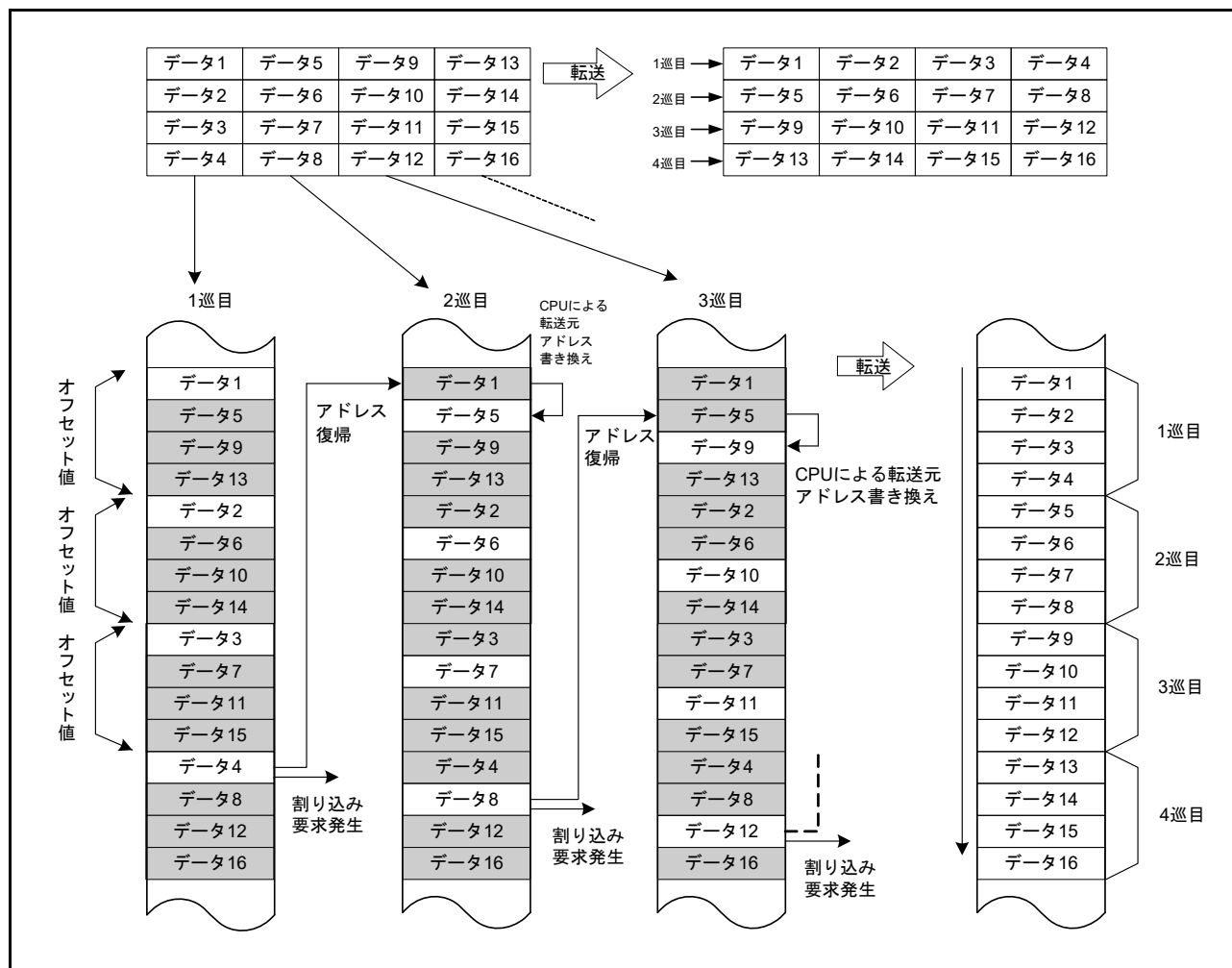
図 16.8 リピート転送モード+オフセット加算によるXY変換動作
