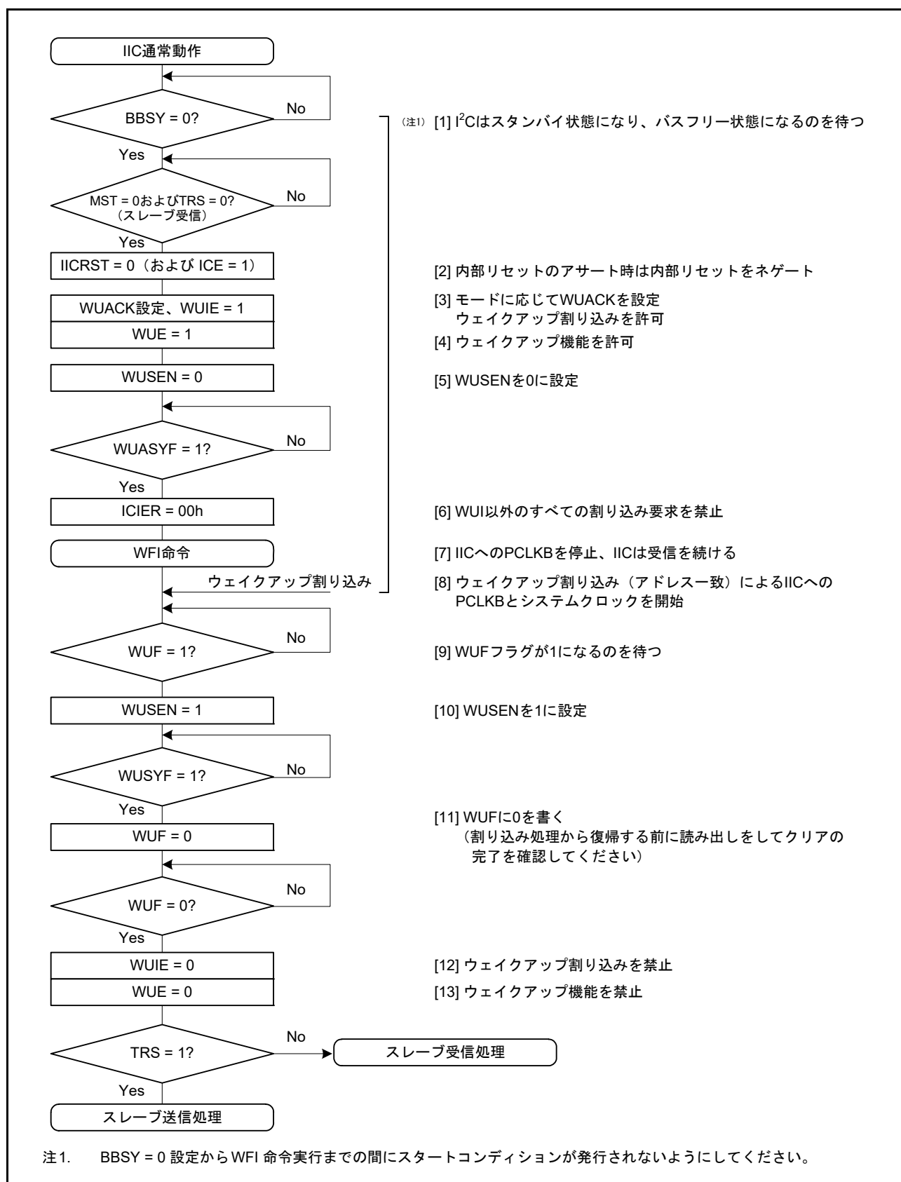
図 29.33 ノーマルウェイクアップモード2の動作例（スレープアドレス一致時のウェイクアップ割り込みによるウェイクアップの場合）
