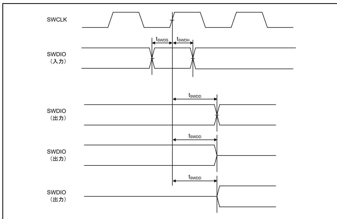
図 48.88 SWD 入出力タイミング
