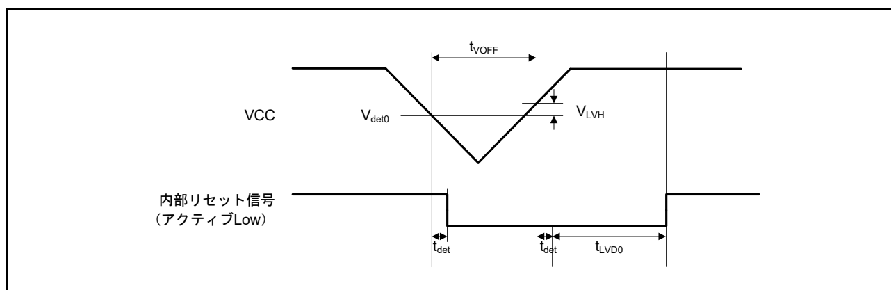
図 48.75 電圧検出回路タイミング ( V_{det0} )
