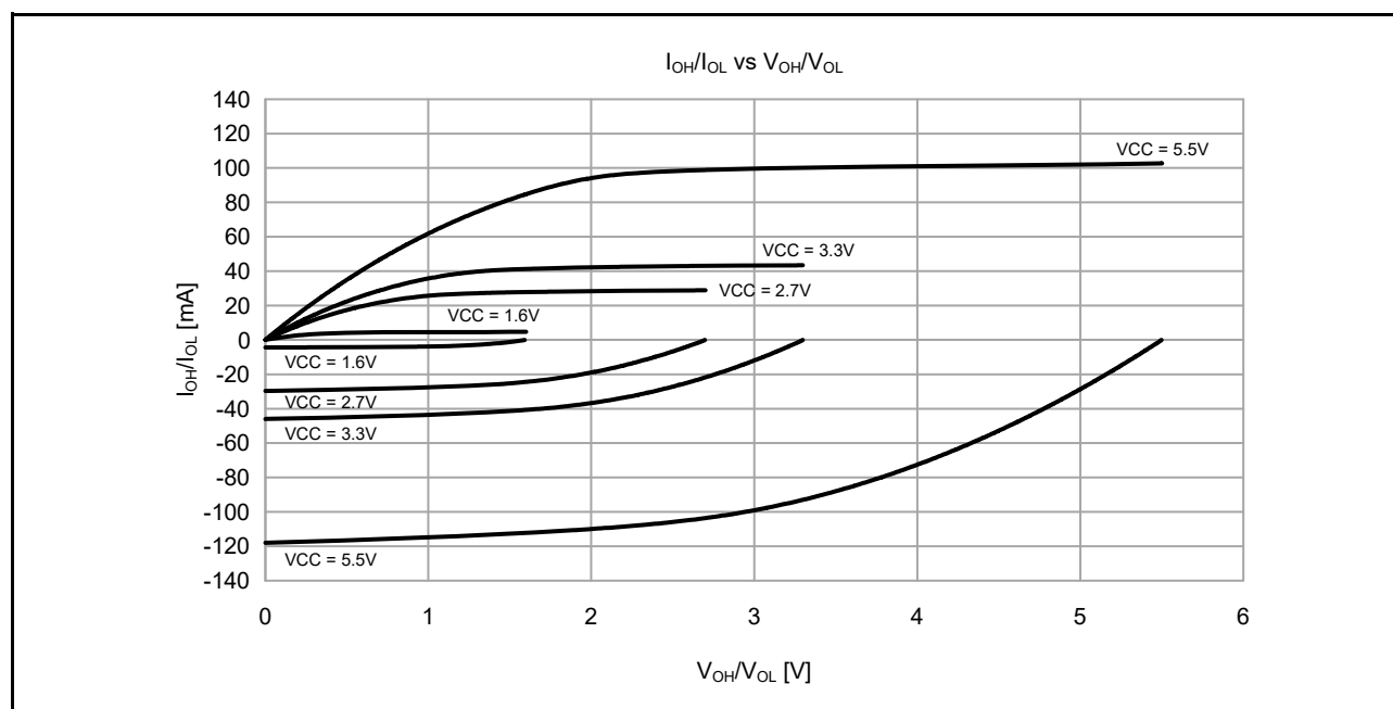
図 48.7 中駆動出力選択時の T_a = 25^\circ\text{C} での V_{OH}/V_{OL} および I_{OH}/I_{OL} 電圧特性 (参考データ)
