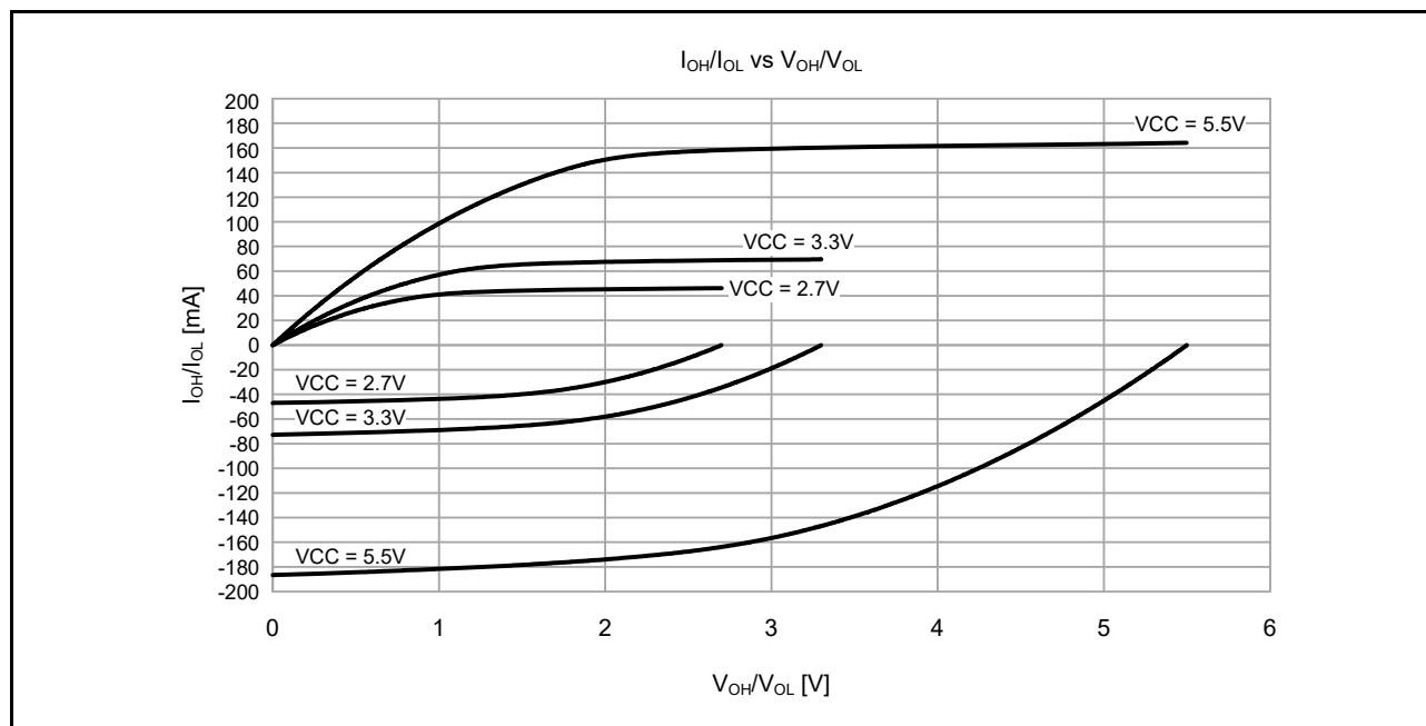
図 48.12 中駆動出力選択時の T_a = 25^\circ\text{C} での V_{OH}/V_{OL} および I_{OH}/I_{OL} 電圧特性 (参考データ)
