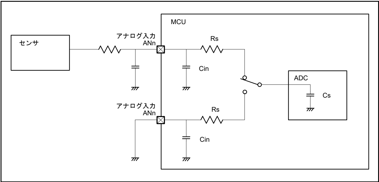
図 48.69 アナログ入力の等価回路
