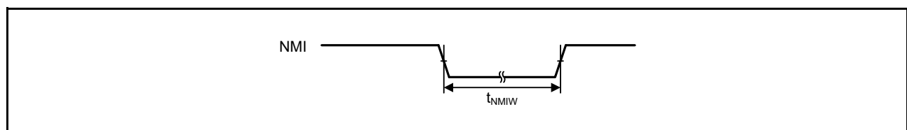
図 48.36 NMI 割り込み入力タイミング
