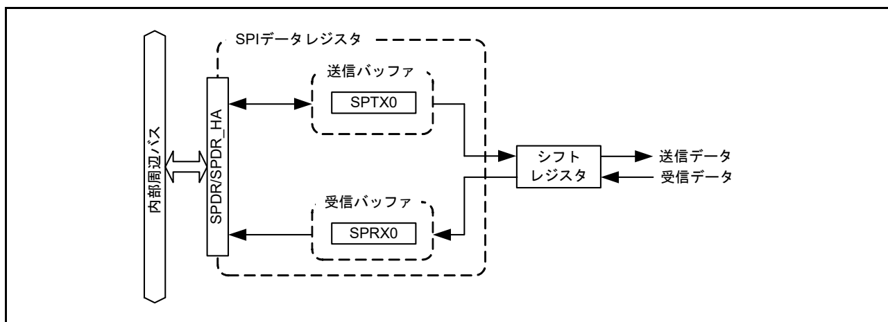
図 31.2 SPDR/SPDR_HA レジスタの構成図
