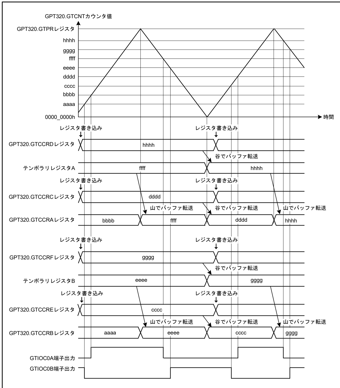
図 22.37 三角波 PWM モード 3 動作例（カウンタスタート時 GTIOC0A 端子 = Low 出力／GTIOC0B 端子 = High 出力、GTCCRA/GTCCRB レジスタのコンペアマッチでトグル出力、周期の終わりで出力保持の場合）
