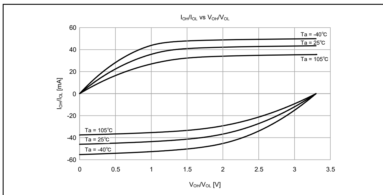
図 48.10 中駆動出力選択時の V_{CC} = 3.3V での V_{OH}/V_{OL} および I_{OH}/I_{OL} 温度特性（参考データ）
