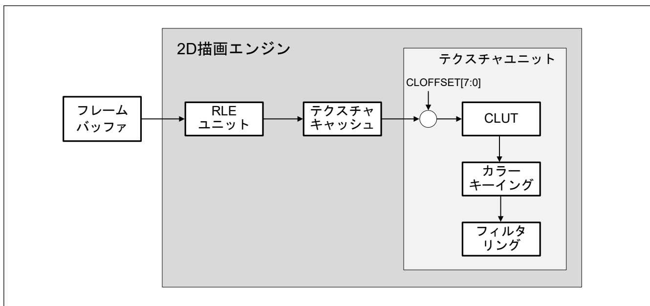
図 55.4 テクスチャデータの処理
