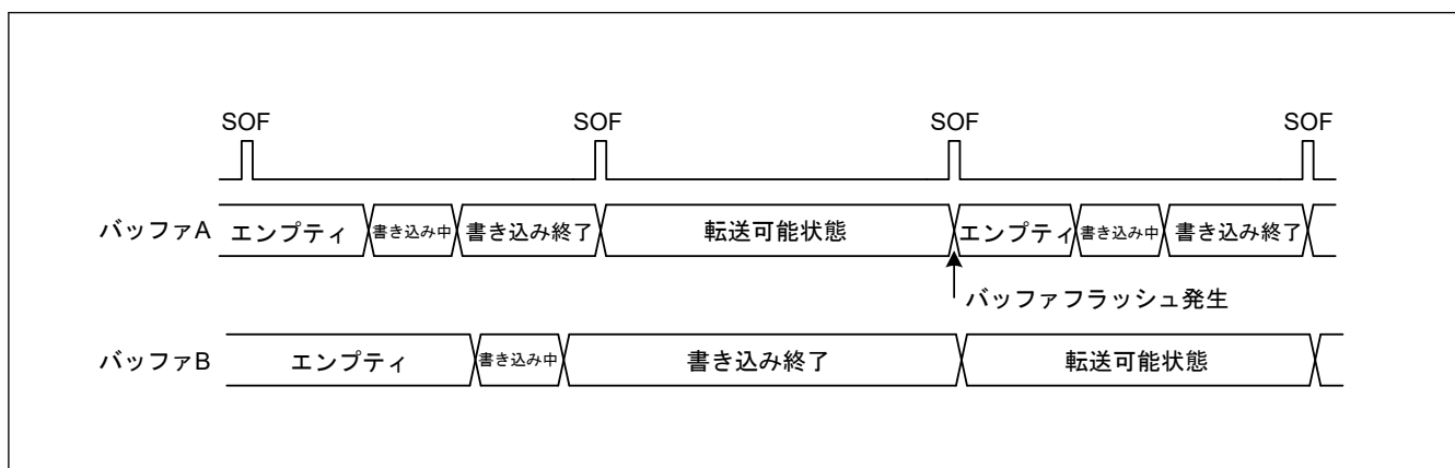
図 30.17 バッファフラッシュ動作例
