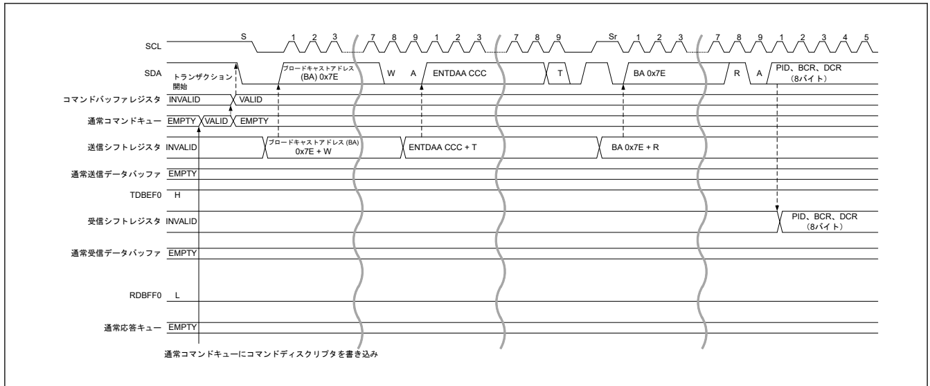
図 33.12 ダイナミックアドレス配置手順 (ENTDAA CCC) タイミング (1/3)
