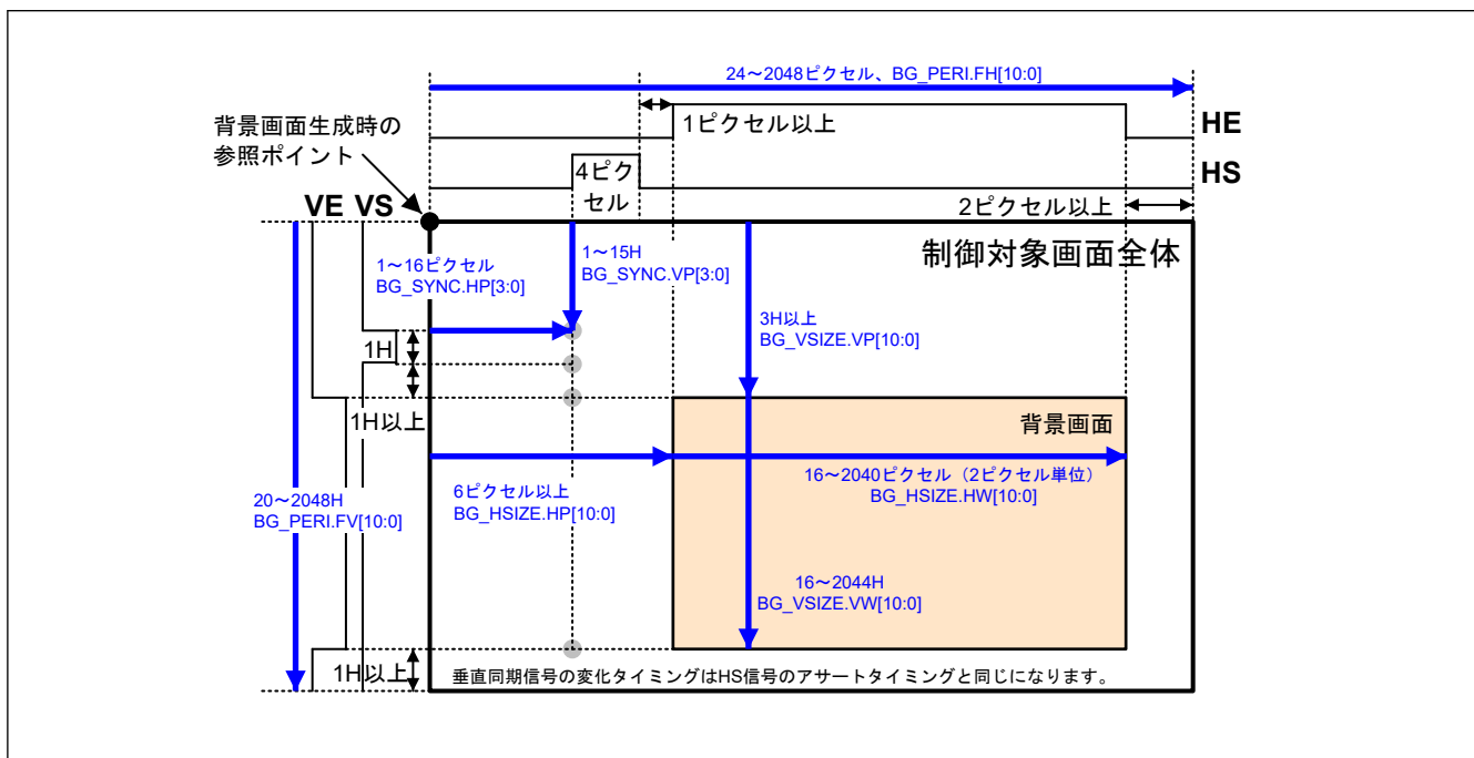
図 56.26 背景画面の定義
