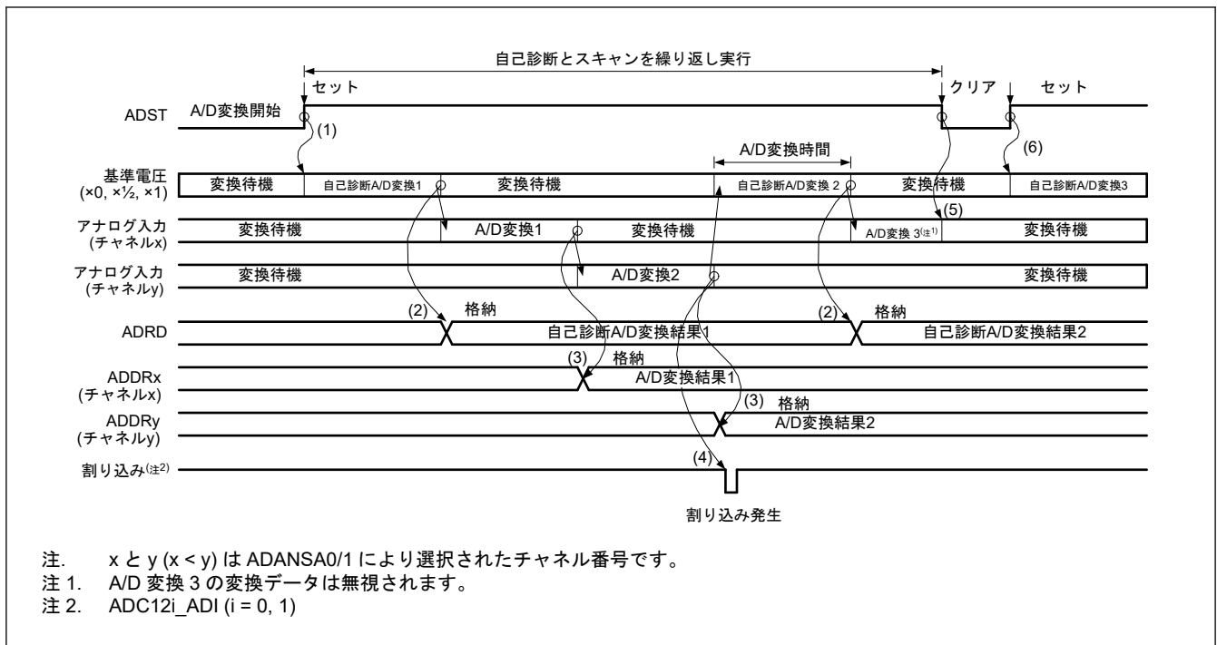
図 45.20 連続スキャンモードの基本動作例 (アナログ入力 (チャンネル x、y) 選択+自己診断)
