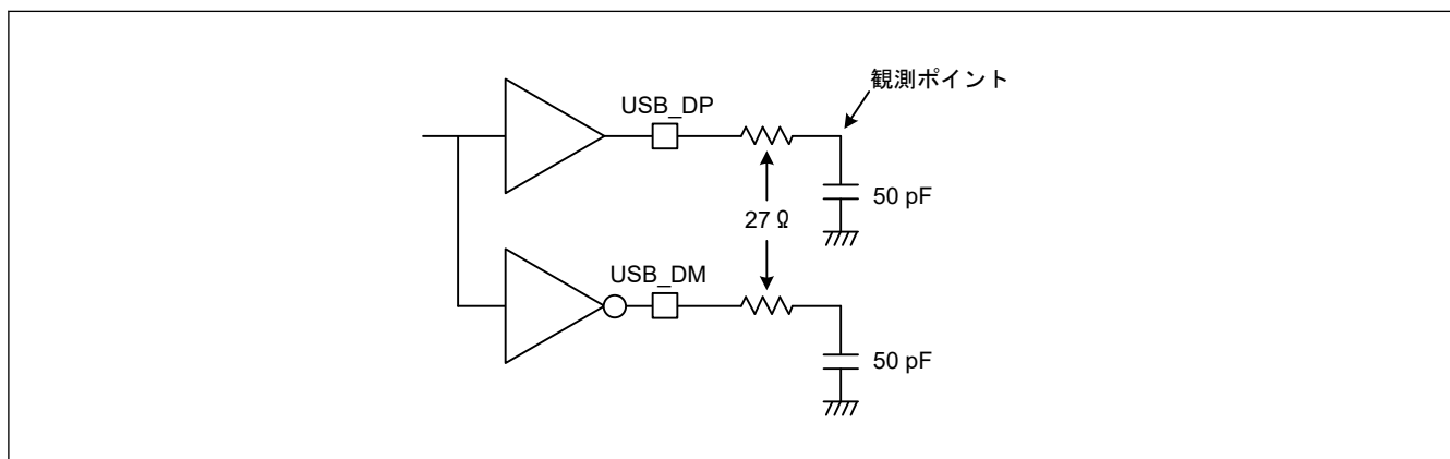
図 60.110 フルスピードモードにおける測定回路
