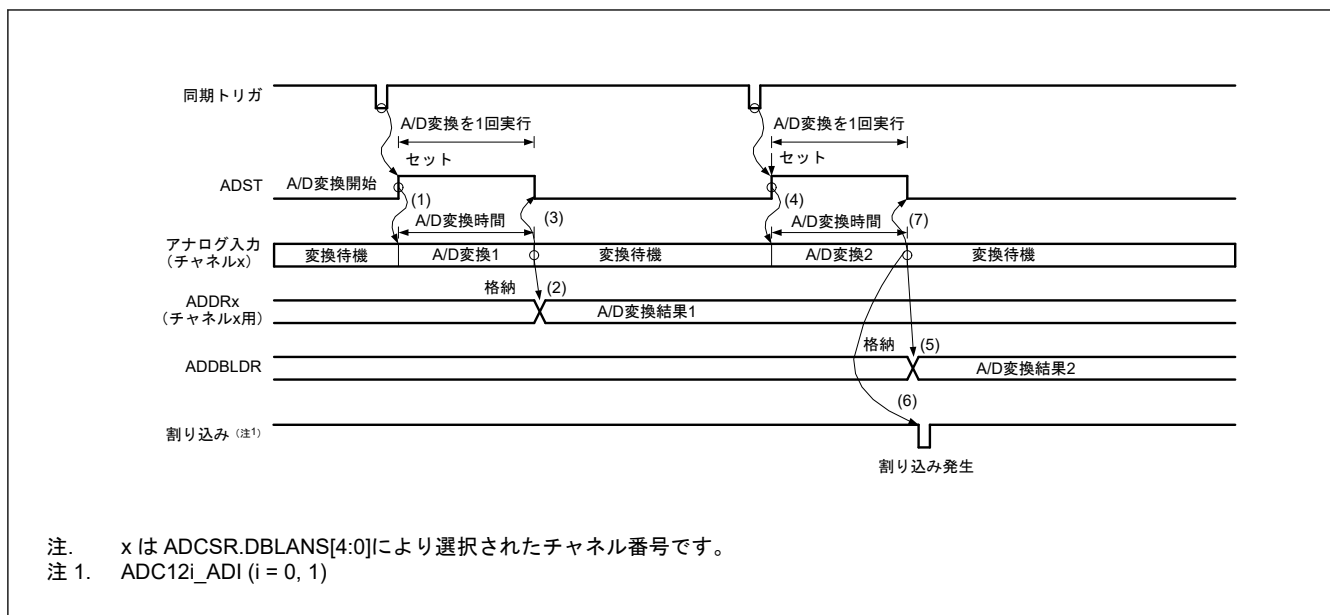
図 45.15 シングルスキャンモードの動作例 (ダブルトリガモード選択、アナログ入力 (チャネル x) を 2 重化)
