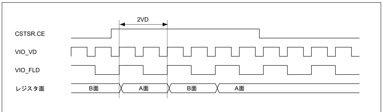
図 53.30 RVS = 0 のときのレジスタ面切り替えタイミング
