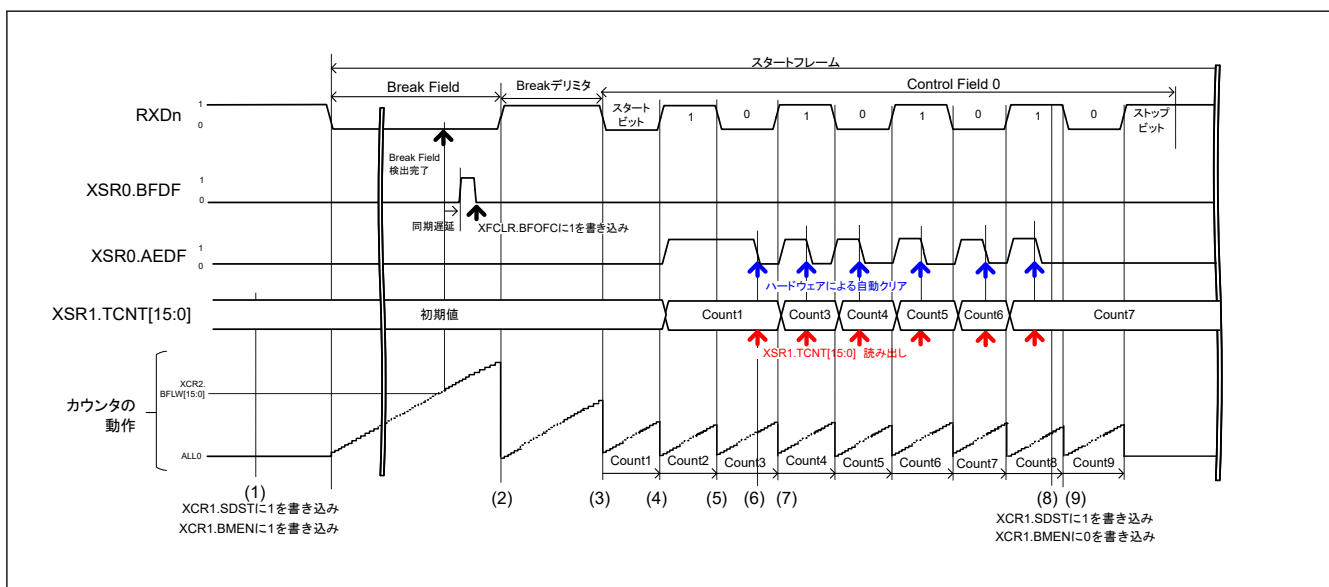
図 31.112 ビットレート測定機能の動作例
