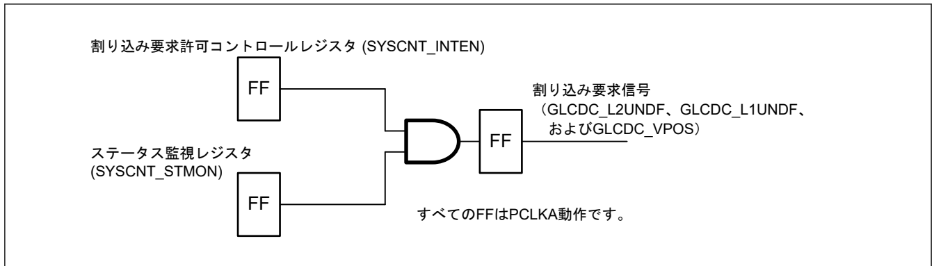
図 56.28 割り込み要求信号生成回路
