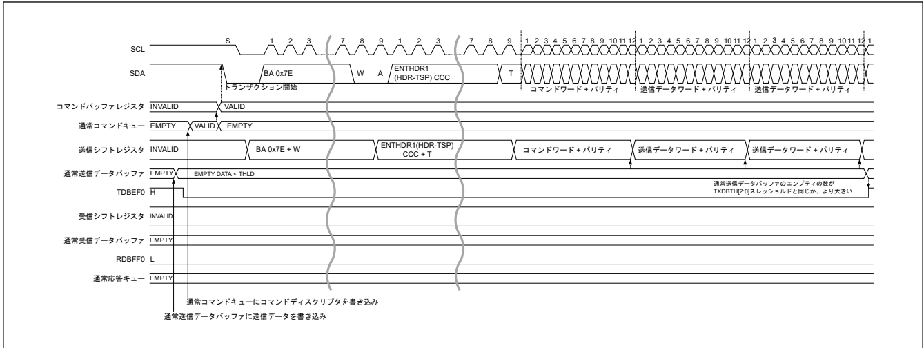
図 33.28 HDR データ書き込み転送 (HDR-TSP、TSL) タイミング (1/2)
