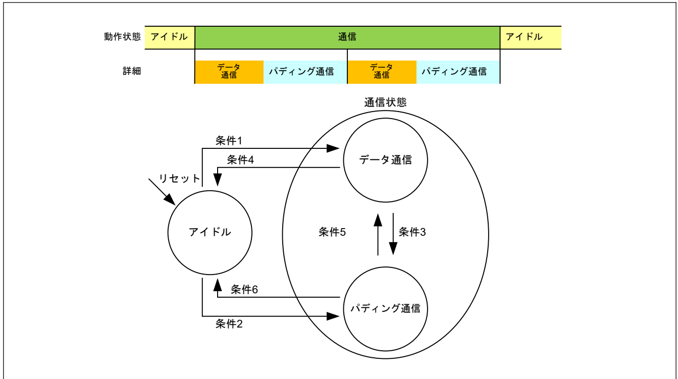
図 39.46 通信状態の遷移
