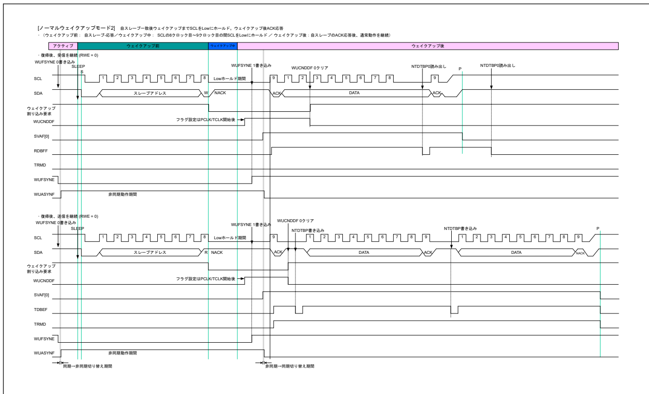
図 33.130 ノーマル WU モード 2 のタイミング
