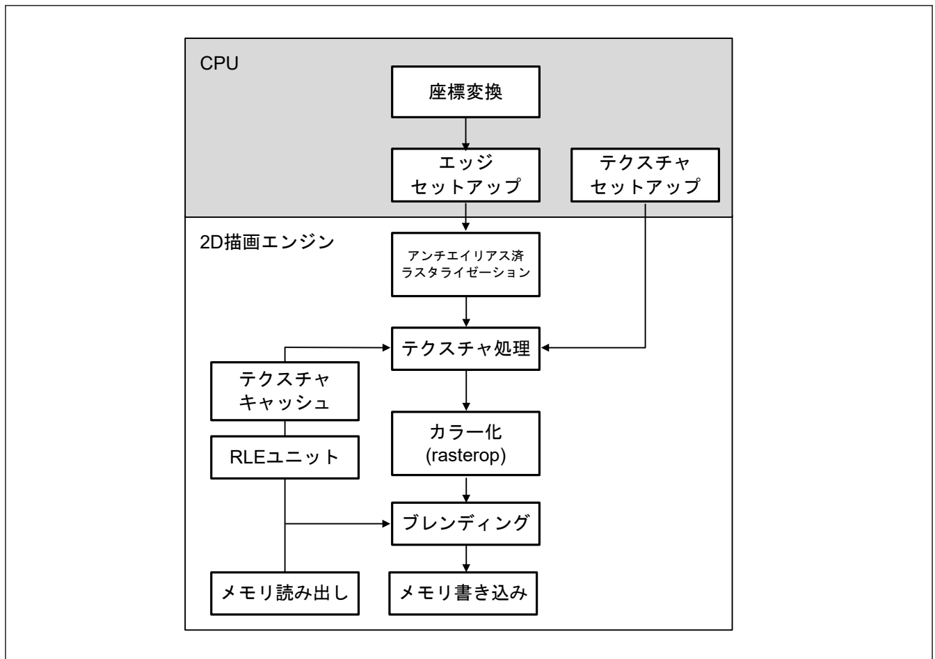
図 55.2 簡略化したレンダリングパイプラインの起動
