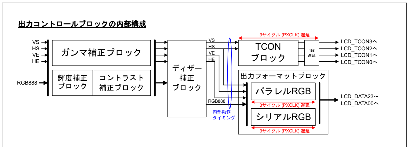
図 56.17 出力コントロールブロックの内部構成
