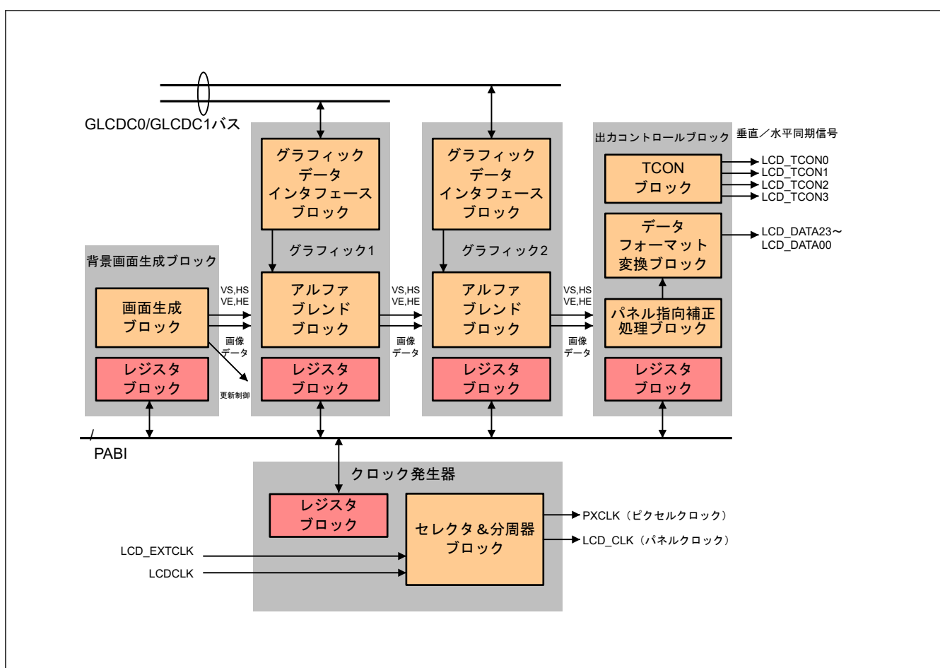
図 56.1 GLCDC のブロック図
