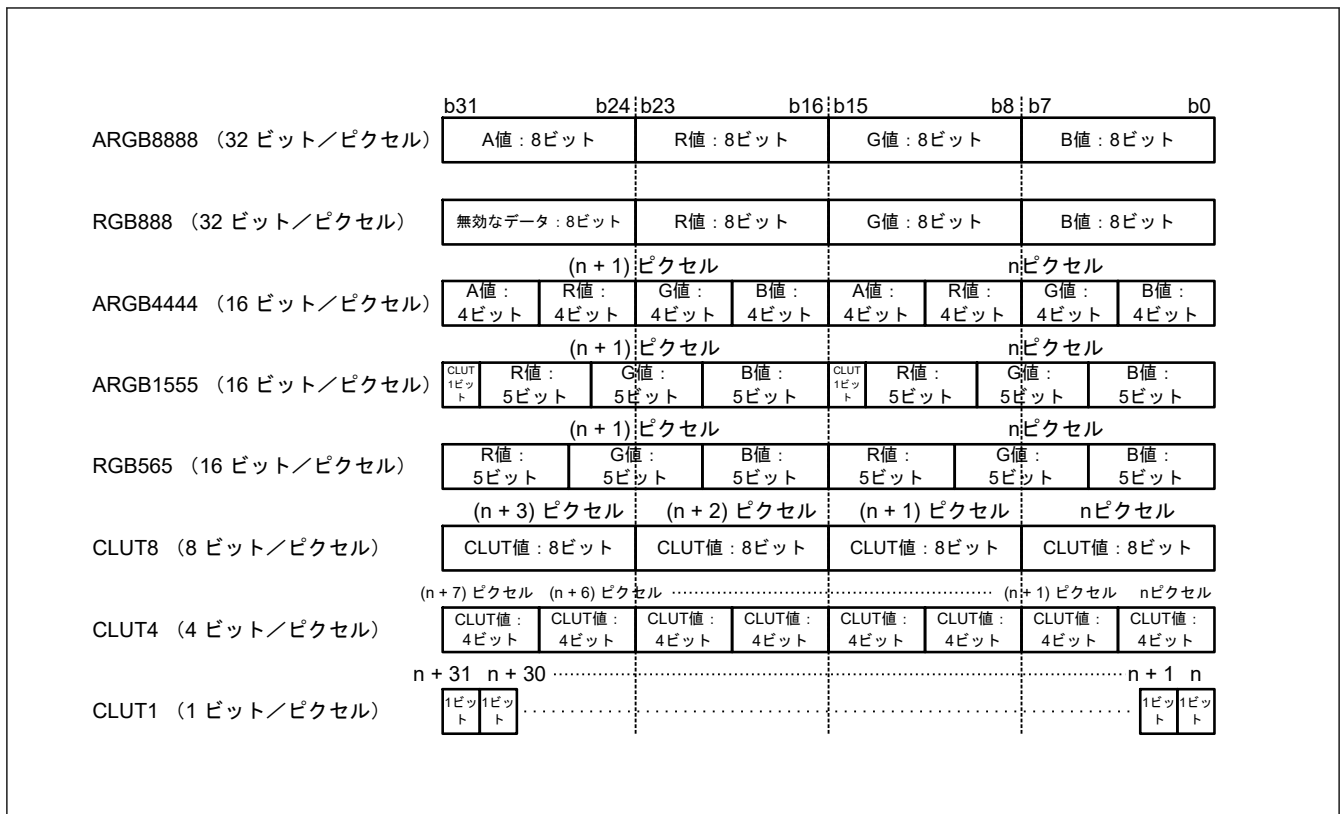
図 56.4 フレームデータのフォーマット
