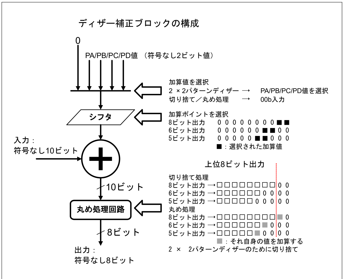
図 56.13 ディザ補正ブロックの構成
