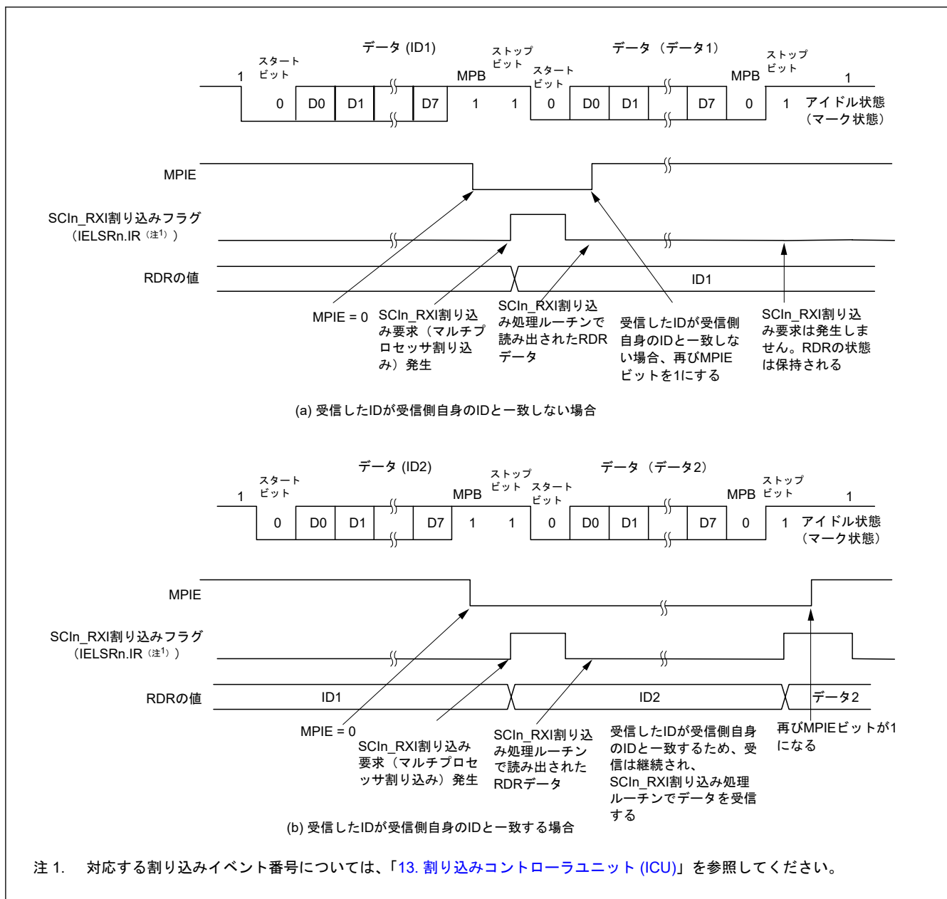
図 31.39 SCIの受信時の動作例 (8ビットデータ/マルチプロセッサビットあり/1ストップビットの場合)
