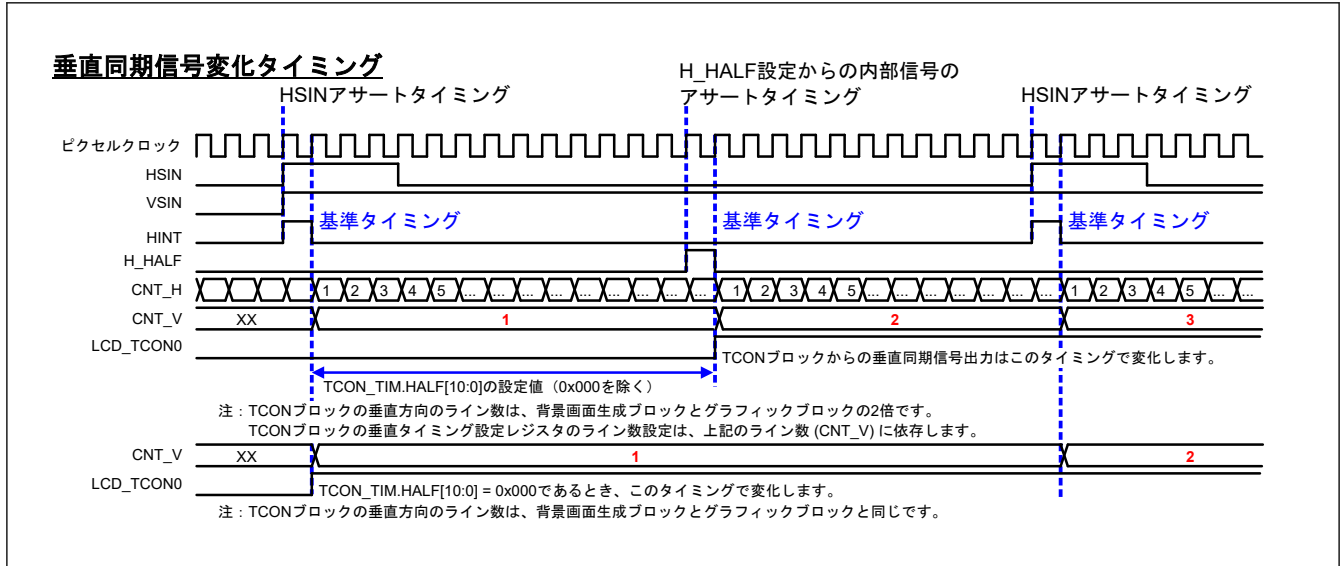
図 56.16 TCON 内の垂直同期信号変化タイミング
