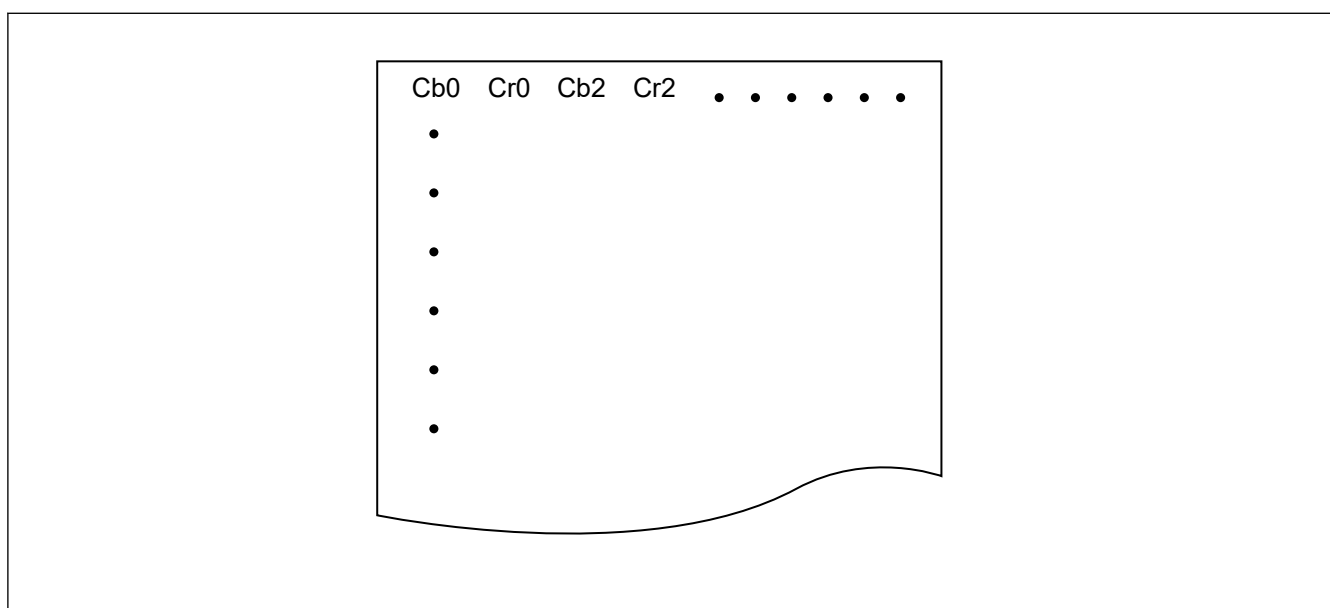
図 53.36 色差成分のメモリ格納イメージ
