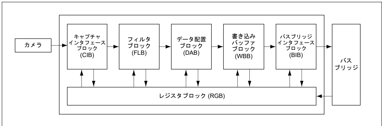
図 53.1 CEU のブロック図
