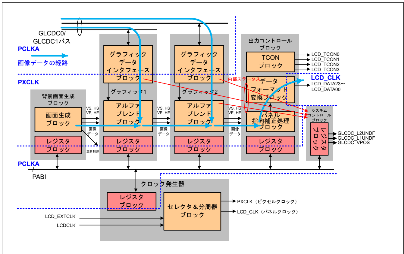
図 56.22 GLCDC の構成
