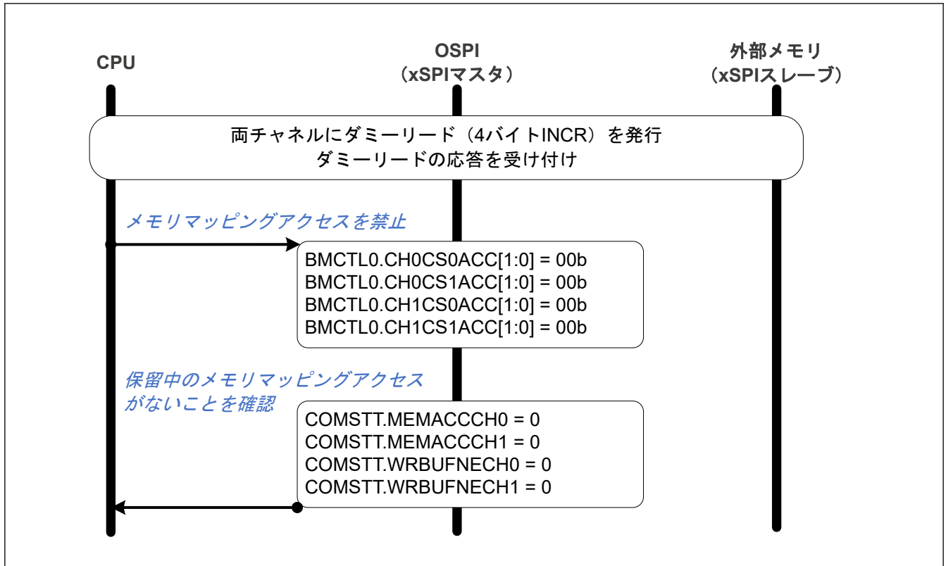
図 37.28 メモリマッピング停止のフロー
