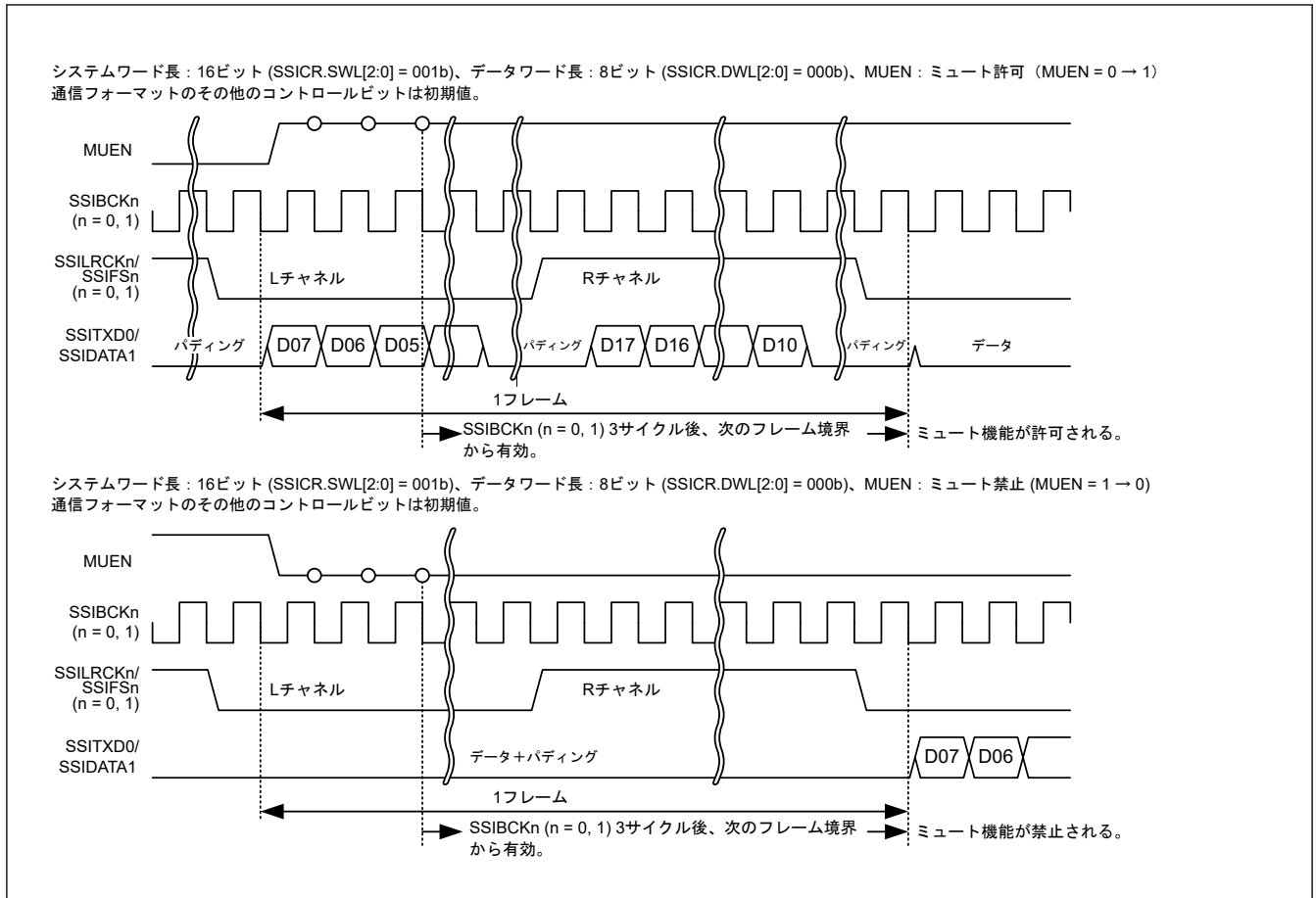
図 39.5 ミュート機能設定時のデータ送信
