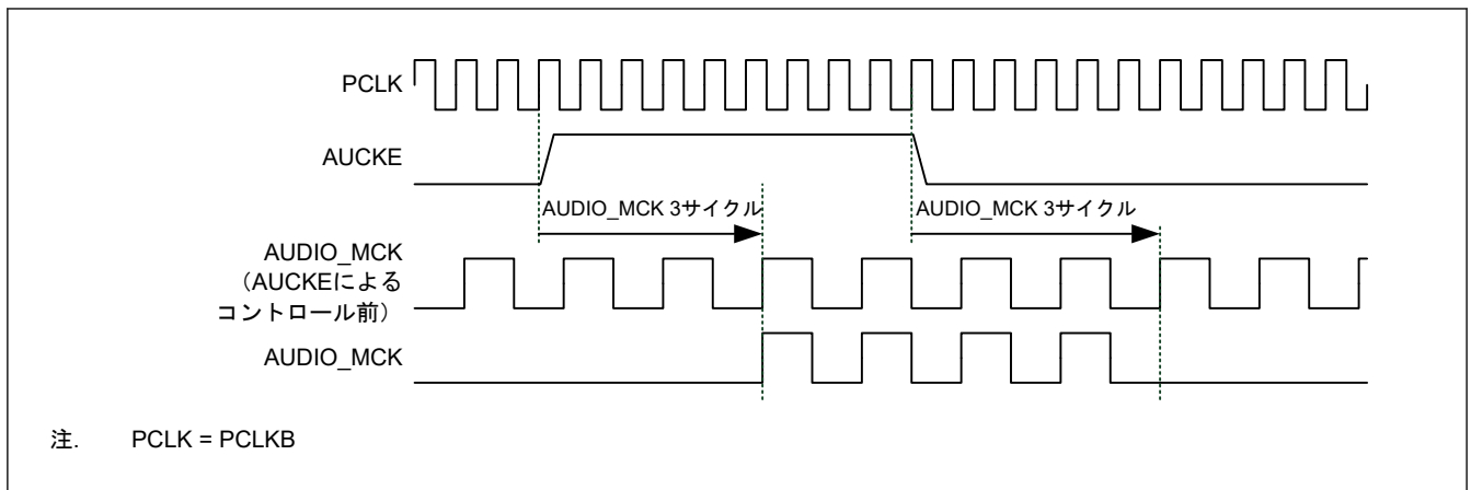
図 39.25 AUDIO_MCK の停止/再開
