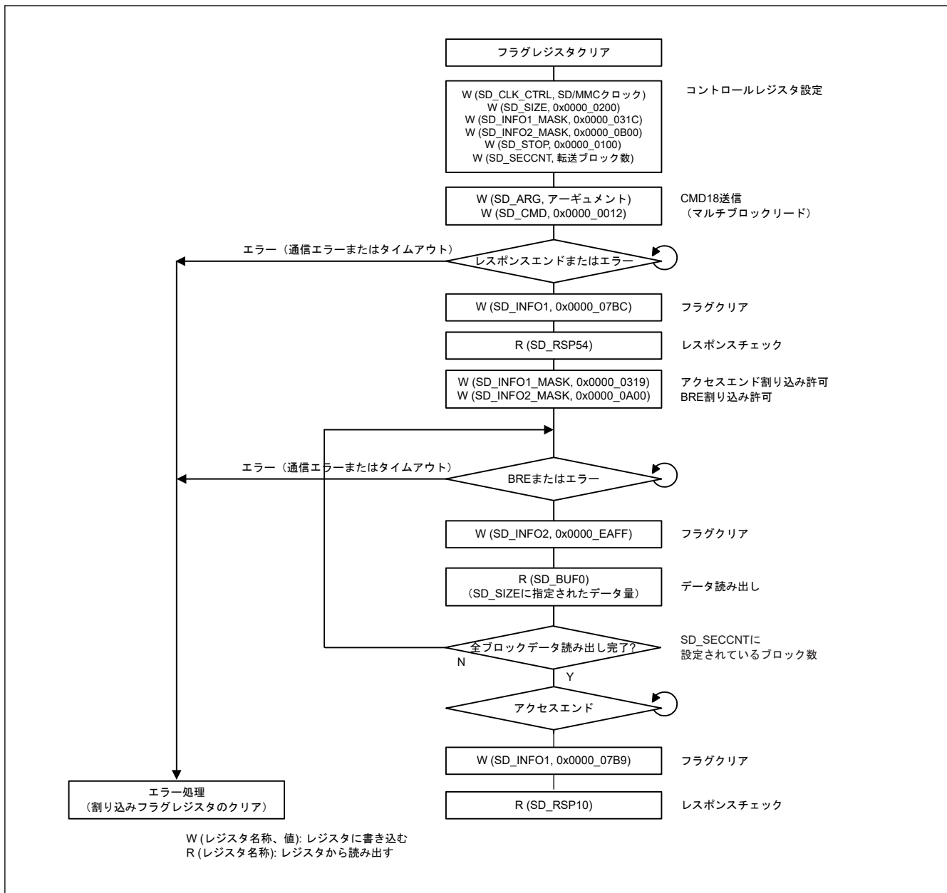
図 40.13 マルチブロックリード動作の例
