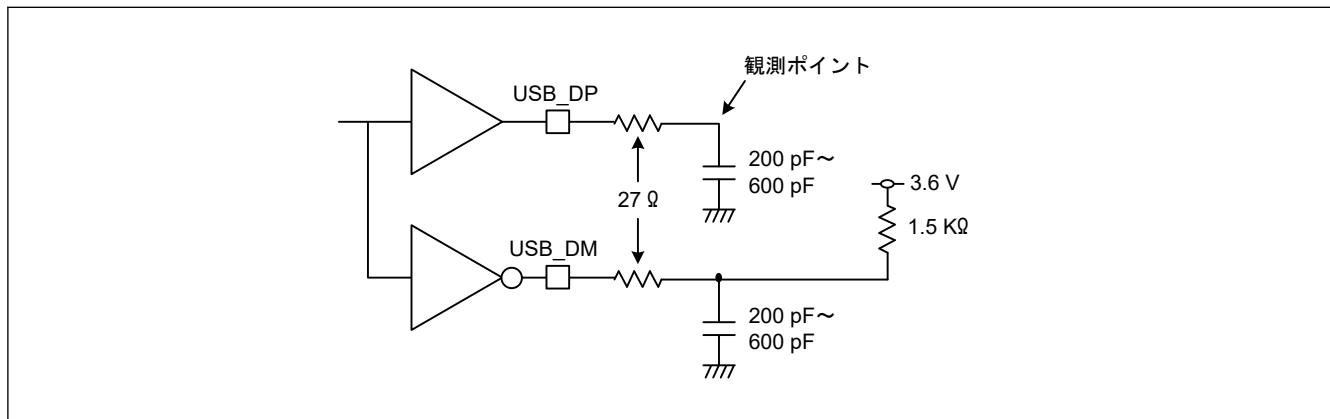
図 60.108 Low-speed モードにおける測定回路
