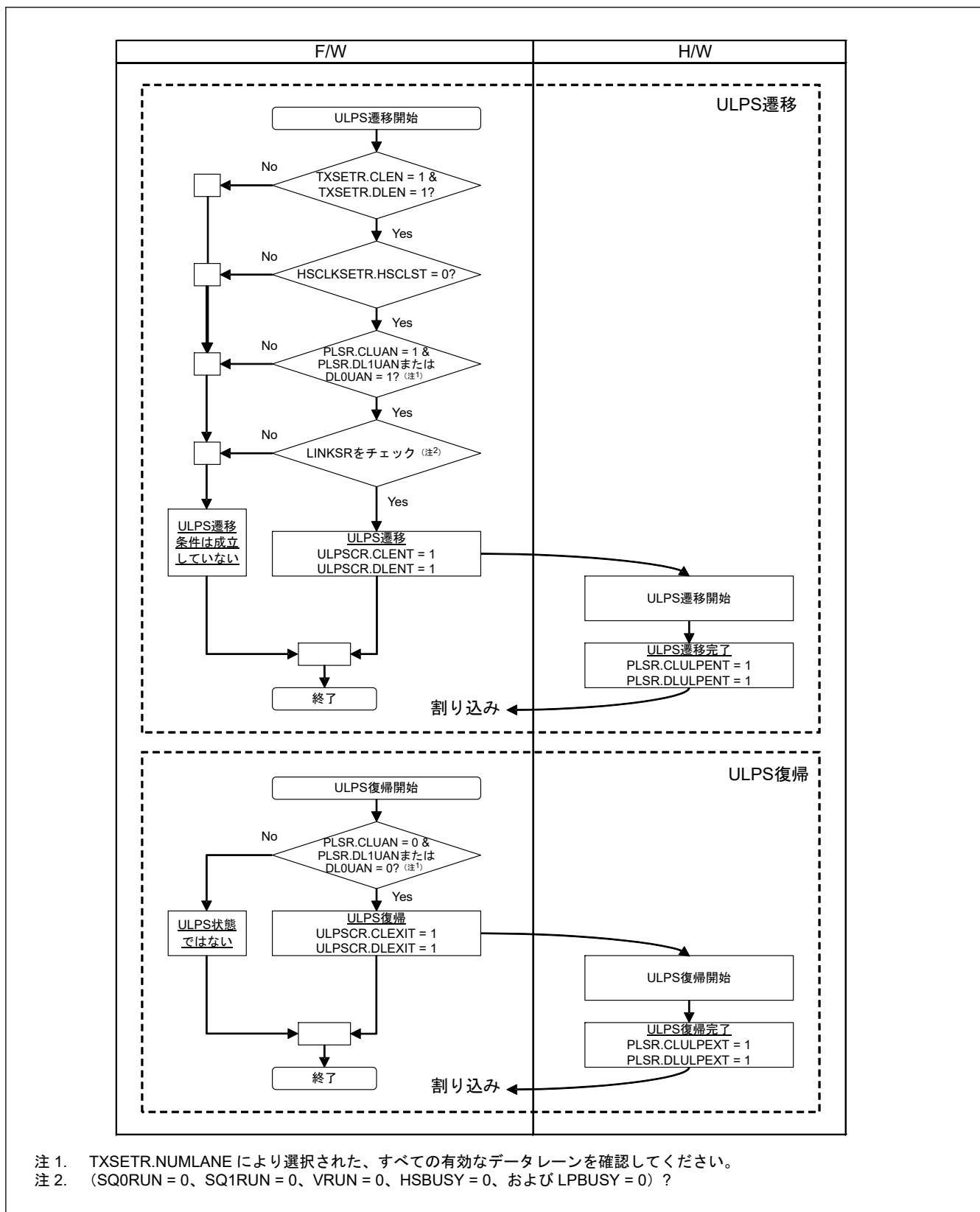
図 58.8 ULPS 遷移/復帰 (クロックレーンとデータレーン)
