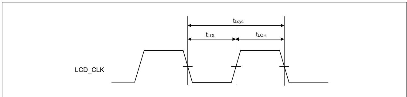
図 60.104 LCD_CLK クロック出力タイミング
