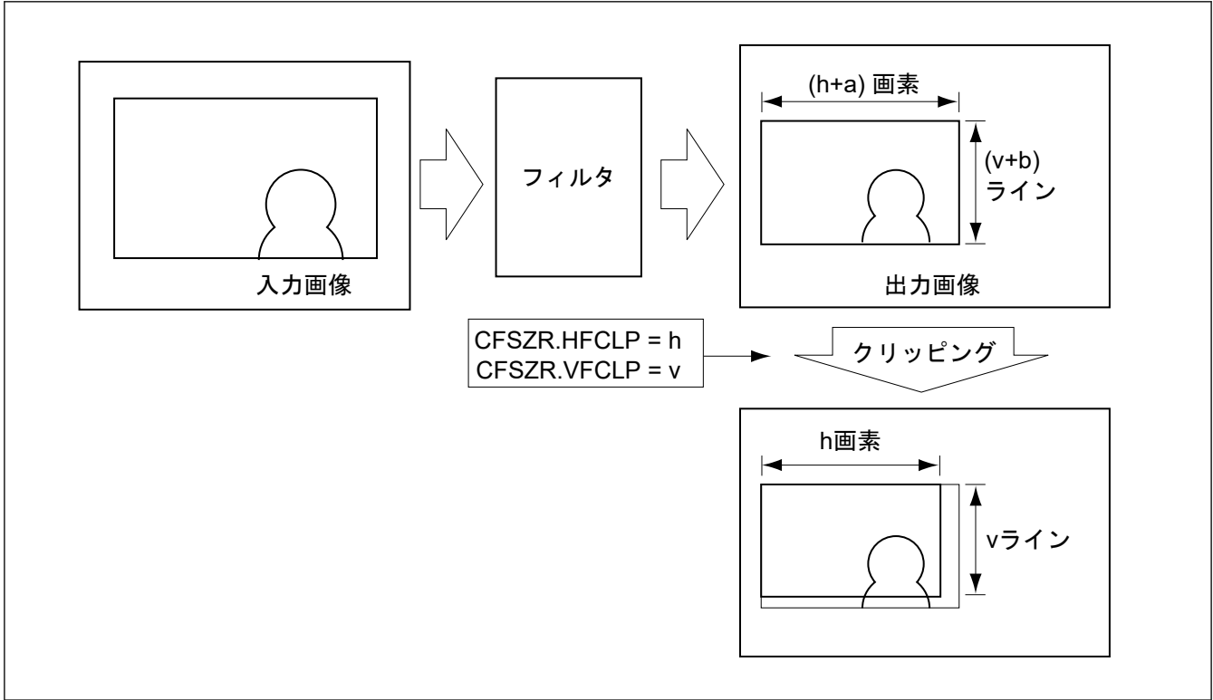
図 53.33 フィルタ出力画像のクリッピング
