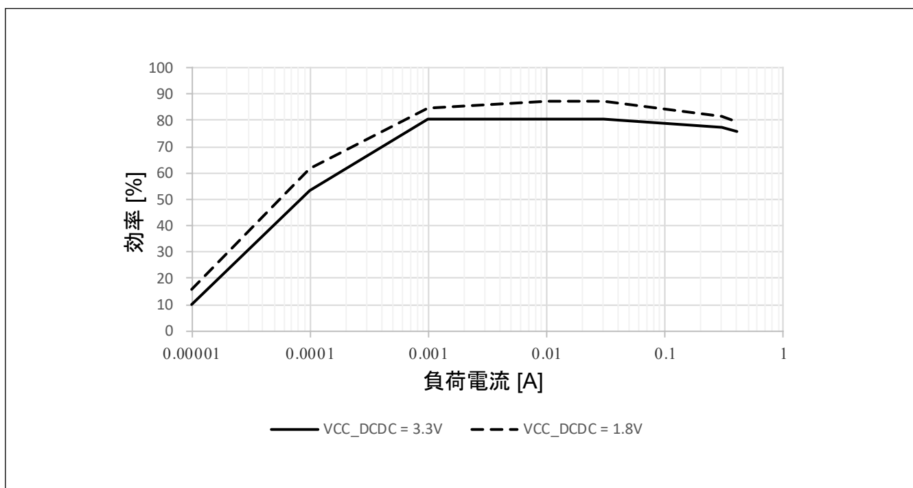
図 60.12 Low-speed モードおよびソフトウェアスタンバイモード、 T_j = 125\text{ }^\circ\text{C} における標準 DCDC 効率 (%) と負荷電流 (A)
