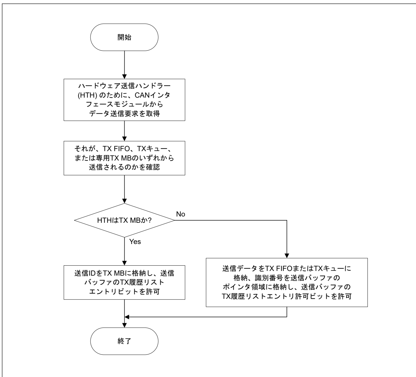
図 34.49 TX履歴リストの準備手順
