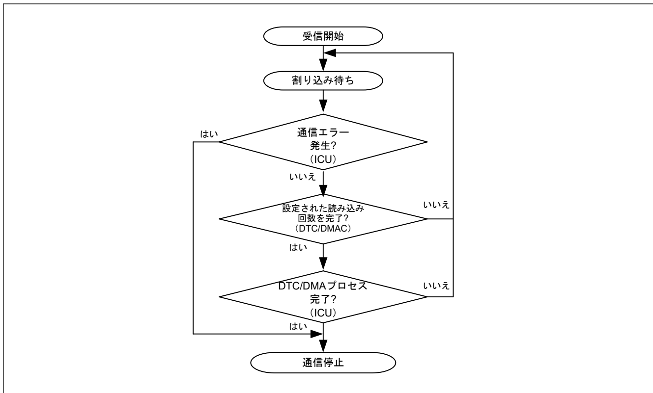
図 39.55 受信手順
