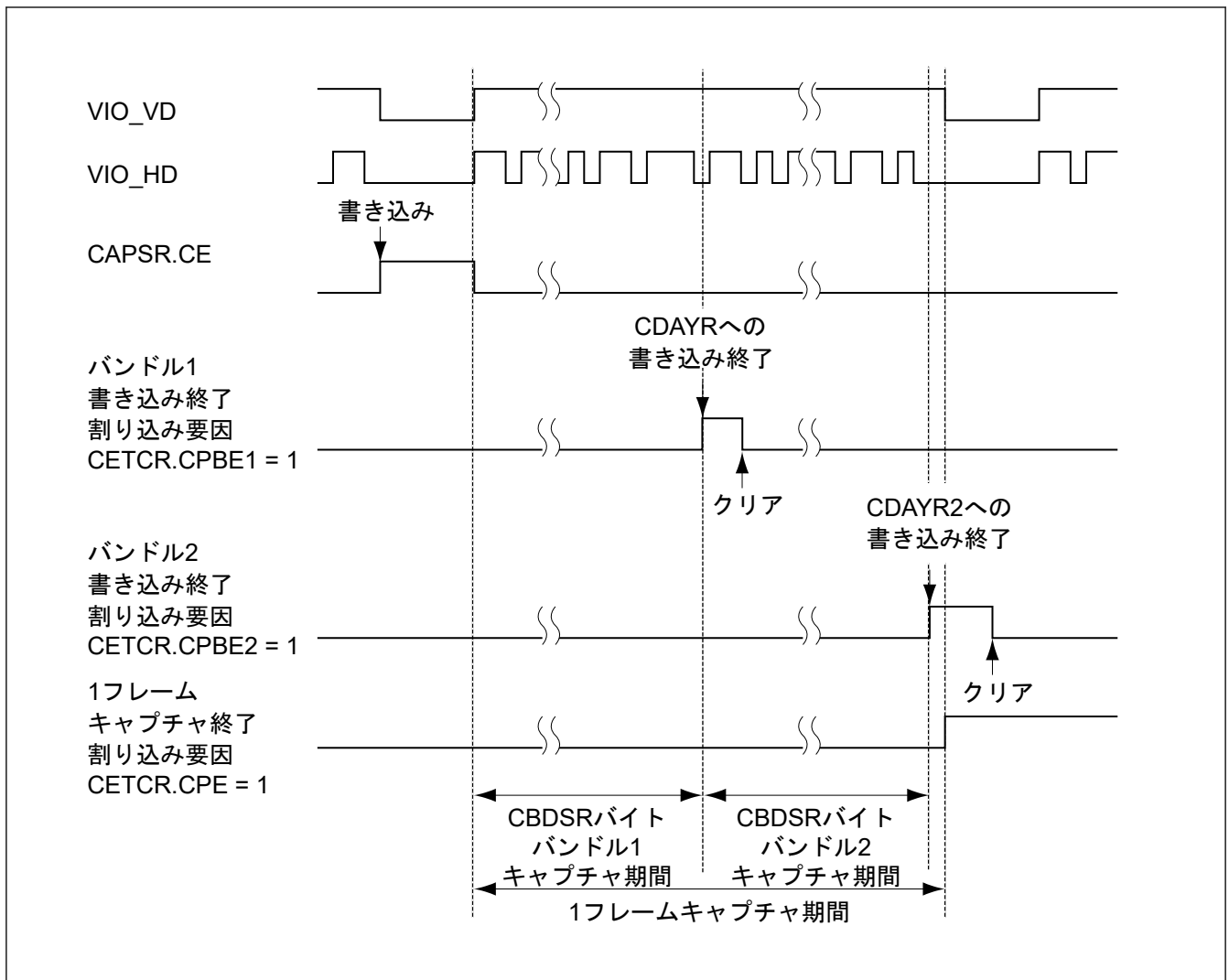
図 53.43 書き込み終了割り込みのタイミング (データインエーブル取り込み時)
