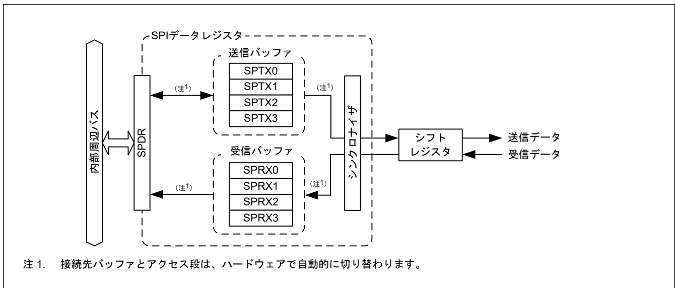
図 36.3 SPDR の構造
