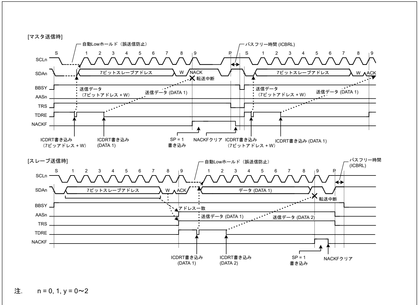
図 32.39 NACK 受信時のデータ転送中断動作 (NACK = 1 の場合)
