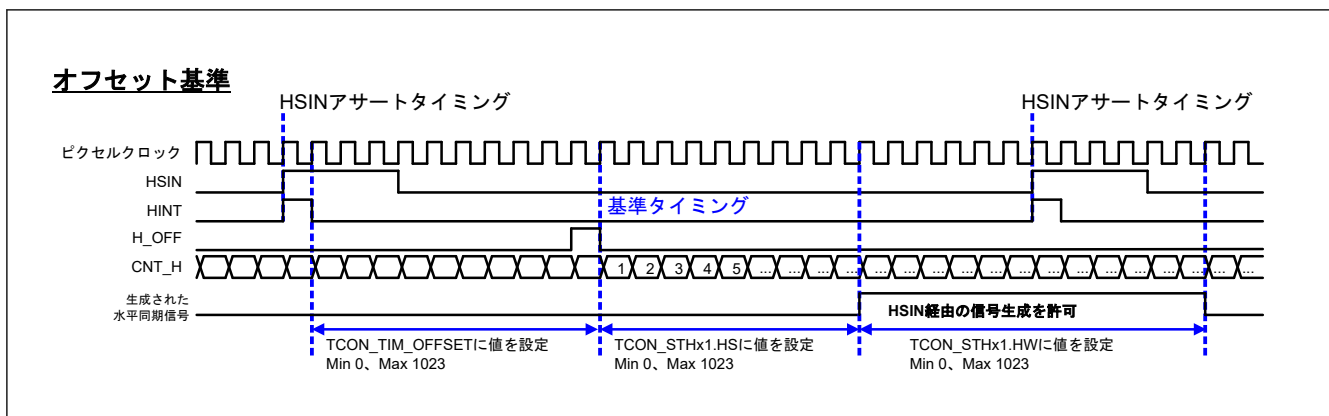
図 56.21 オフセットに基づく水平同期信号生成
