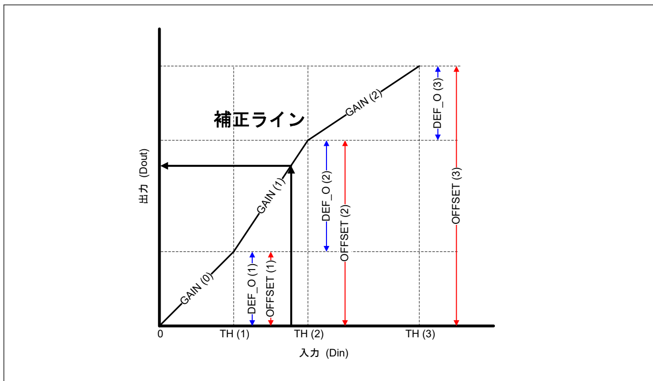
図 56.12 ガンマ補正値の計算
