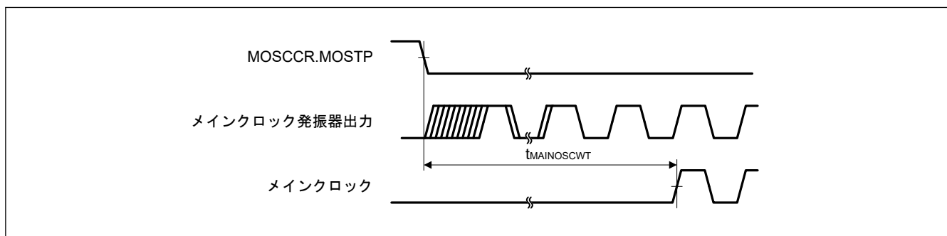
図 60.17 メインクロック発振開始タイミング
