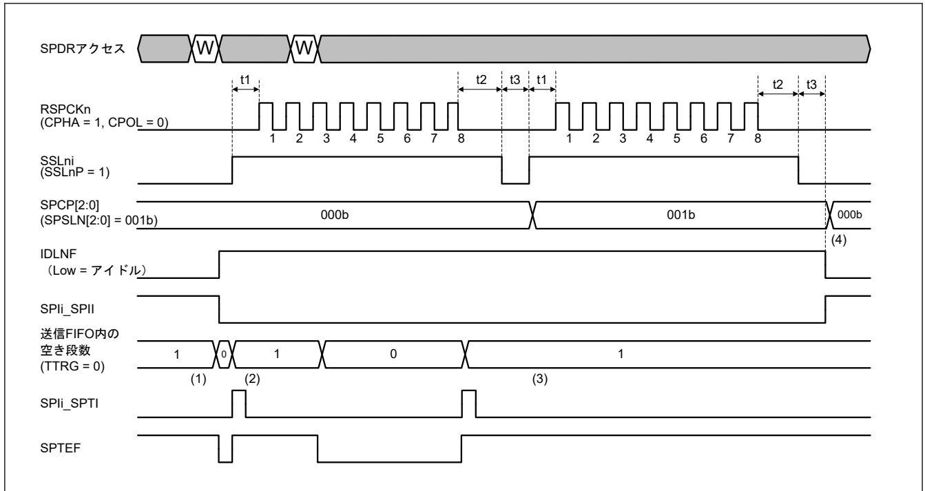
図 36.34 アイドル割り込み動作の例 (マスターモード/Motorola-SPI)
