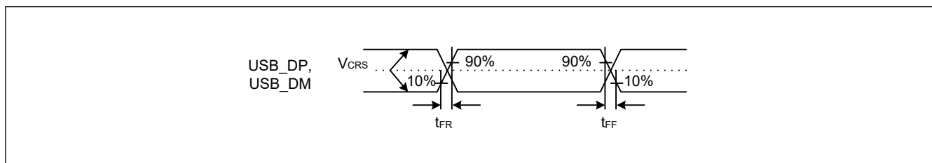
図 60.109 フルスピードモードにおける USB_DP、USB_DM の出力タイミング
