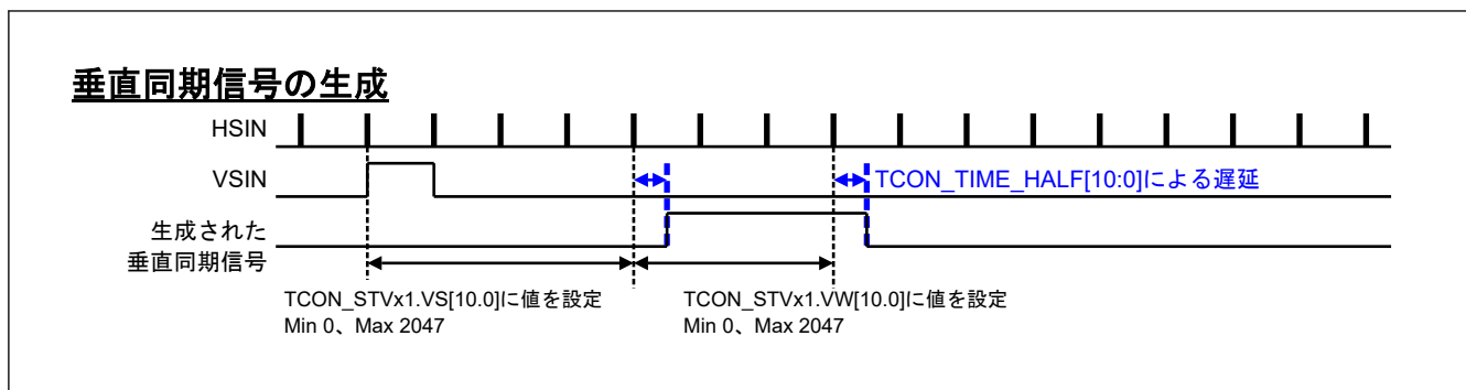
図 56.18 垂直同期信号の生成
