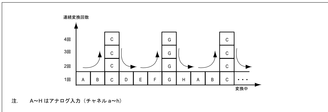
図 45.3 ADADC.ADC[2:0] = 011b および ADADS0/1 によるアナログ入力 C と G を 1 に選択時のスキャン変換シーケンス
