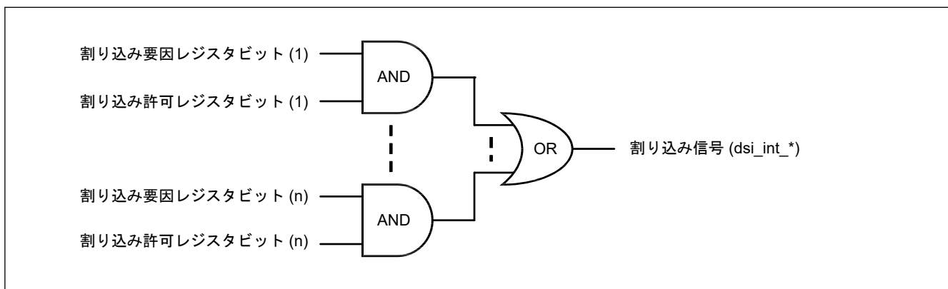
図 58.3 割り込み信号出力
