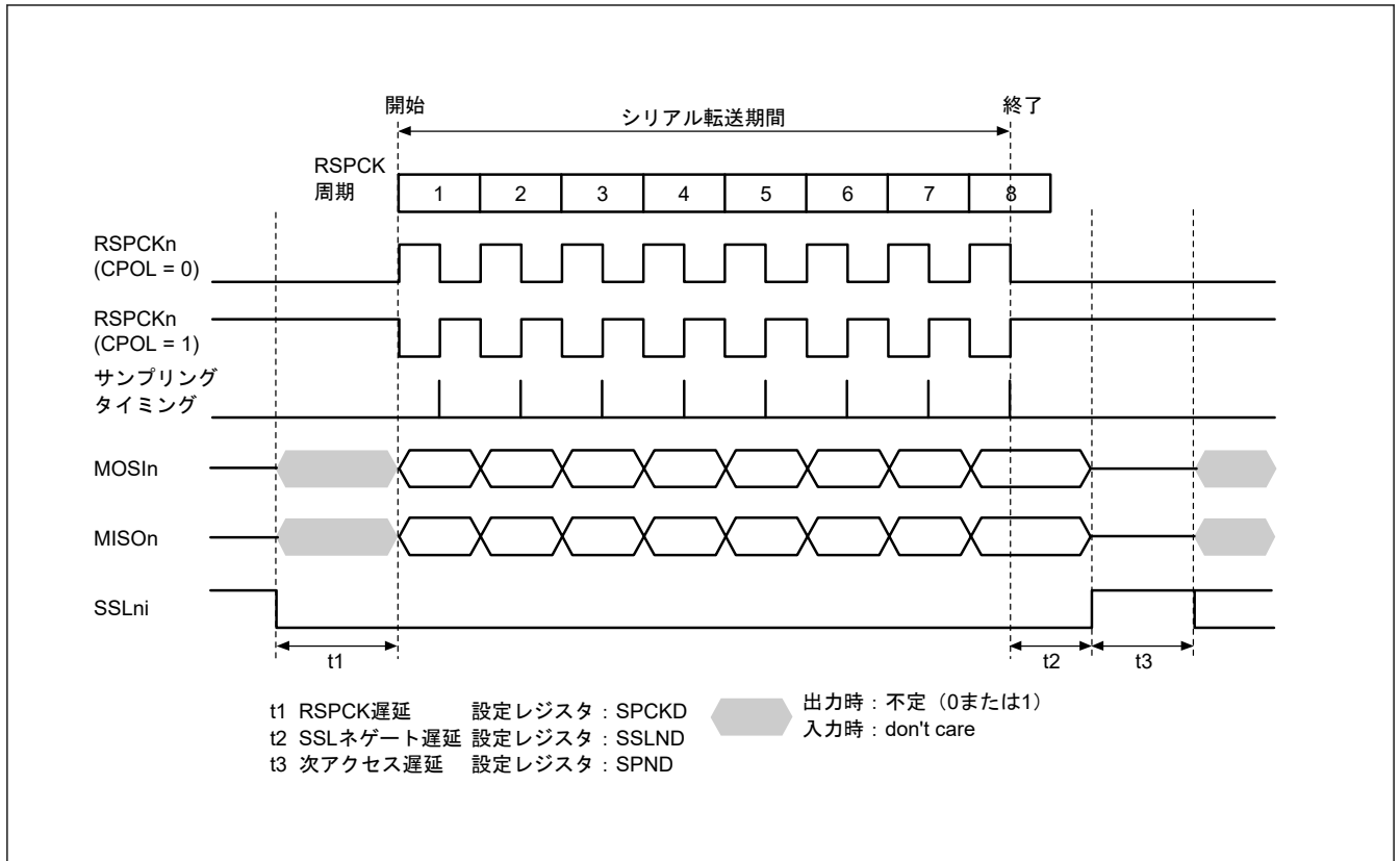
図 36.28 CPHA = 1、SPFRF = 0 の場合の SPI 転送フォーマット
