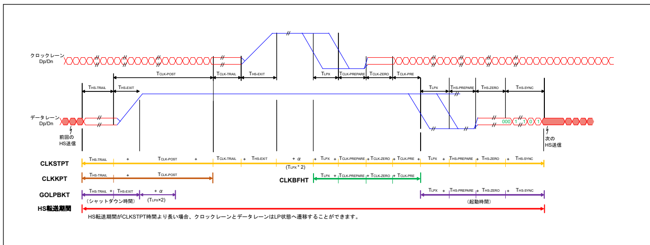
図 58.1 クロックレーンでの LP モードの最小継続時間
