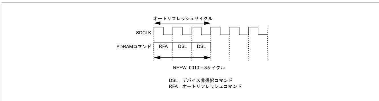
図 14.40 オートリフレッシュサイクルのタイミング例 (1)
