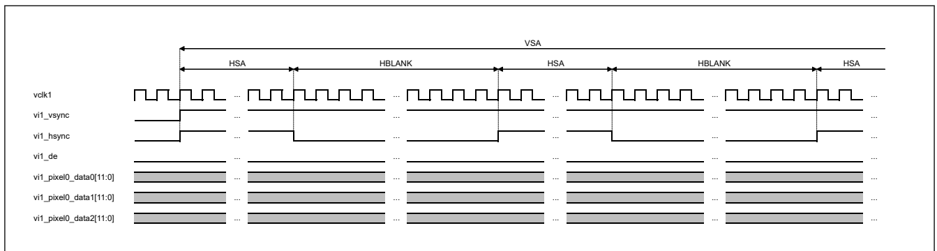
図 58.10 VSA 開始 (と VFP 終了)
