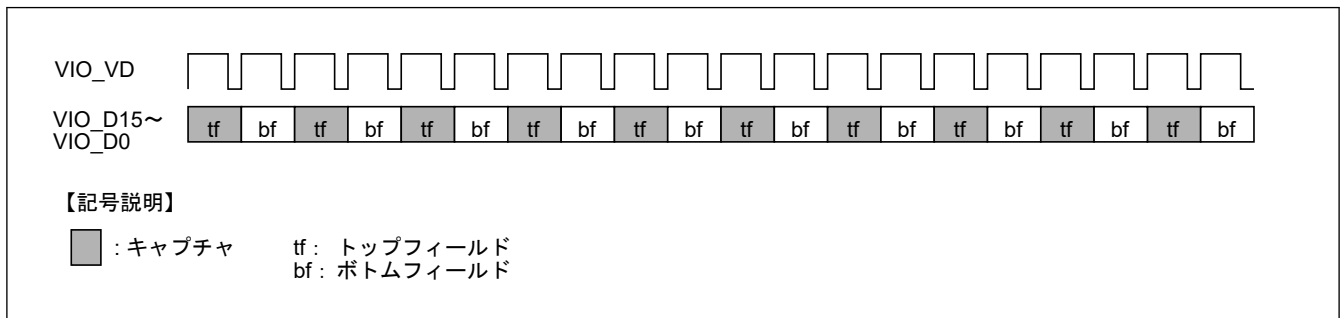
図 53.27 インターレース入力方式での片フィールド連続キャプチャ（起動直後の画像がトップフィールドの場合 (FCI[1:0] = 00b)
