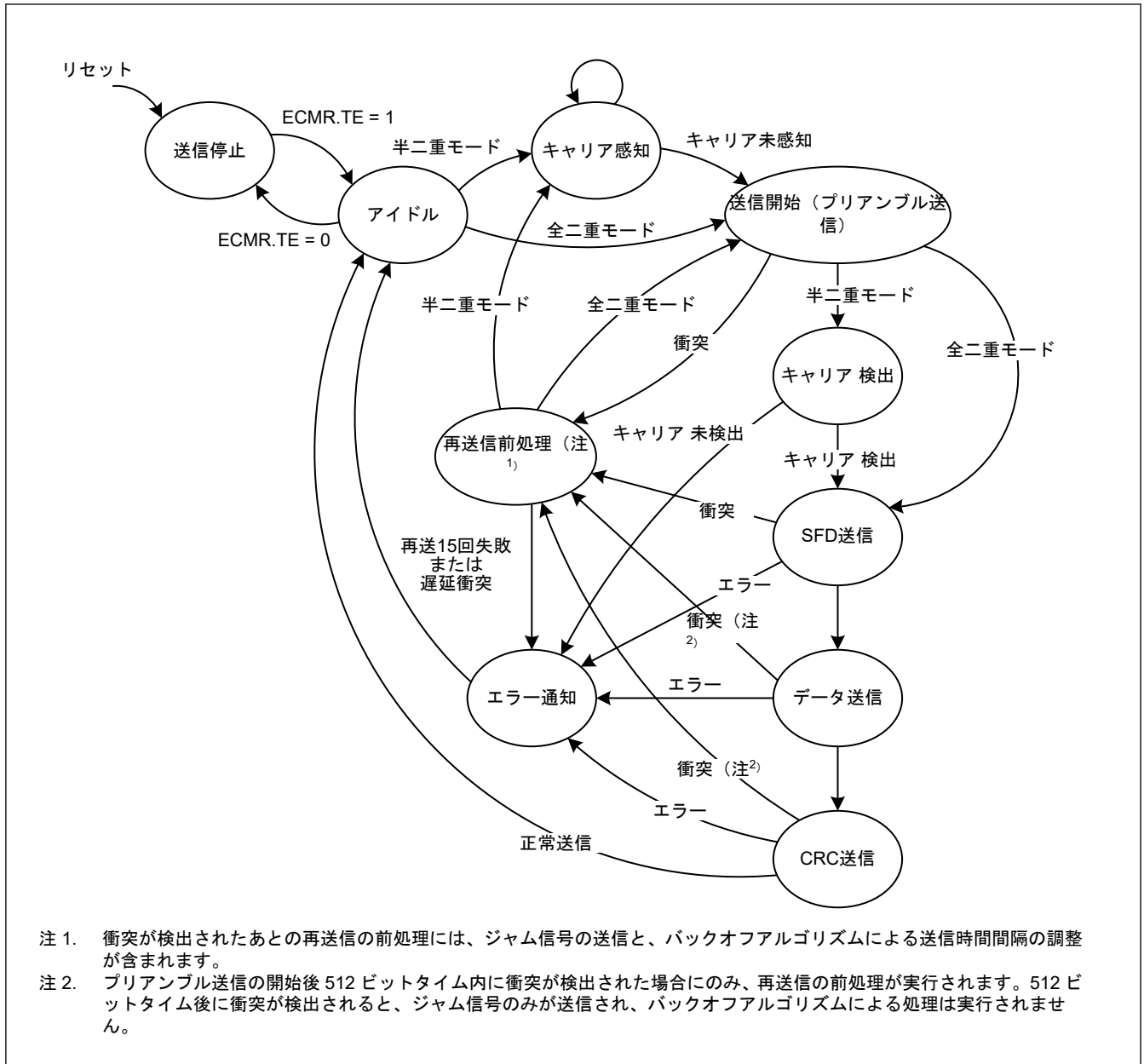
図 27.4 ETHERC 送信部の状態遷移
