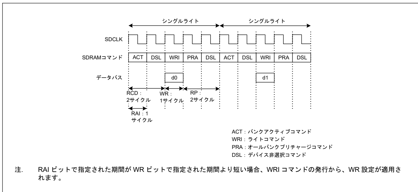
図 14.58 シングルライトタイミング例 (2)
