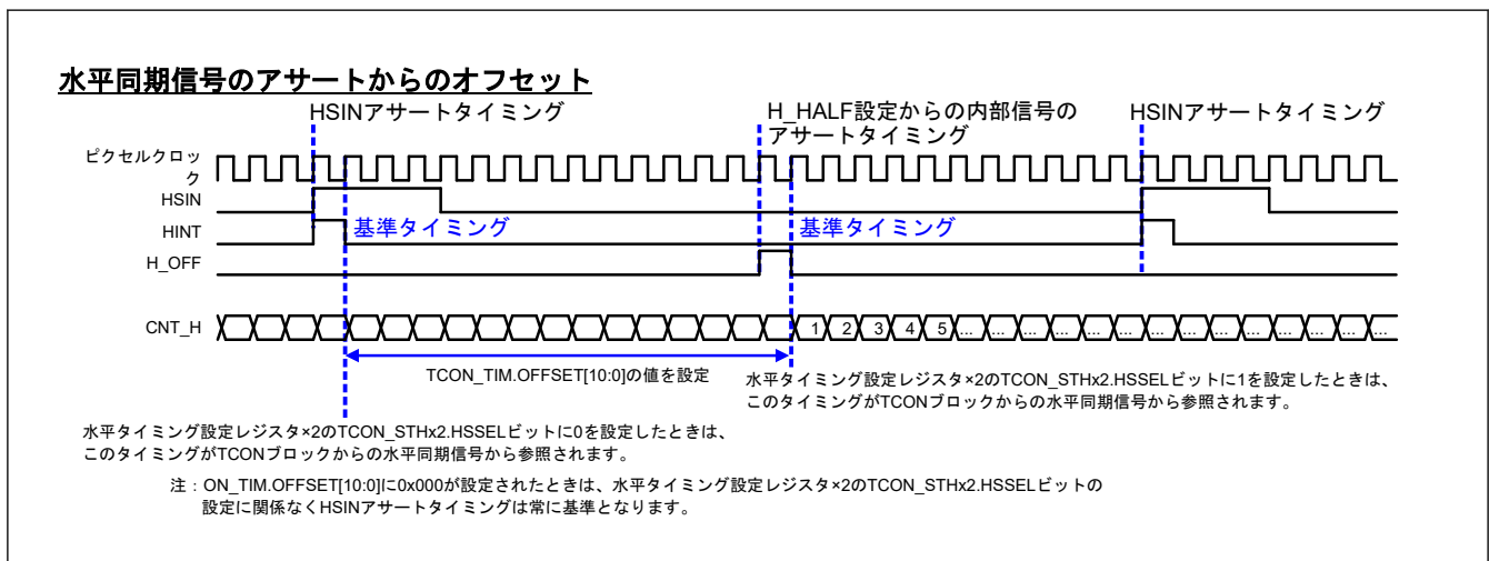
図 56.15 TCON 内水平同期信号生成用参照タイミング
