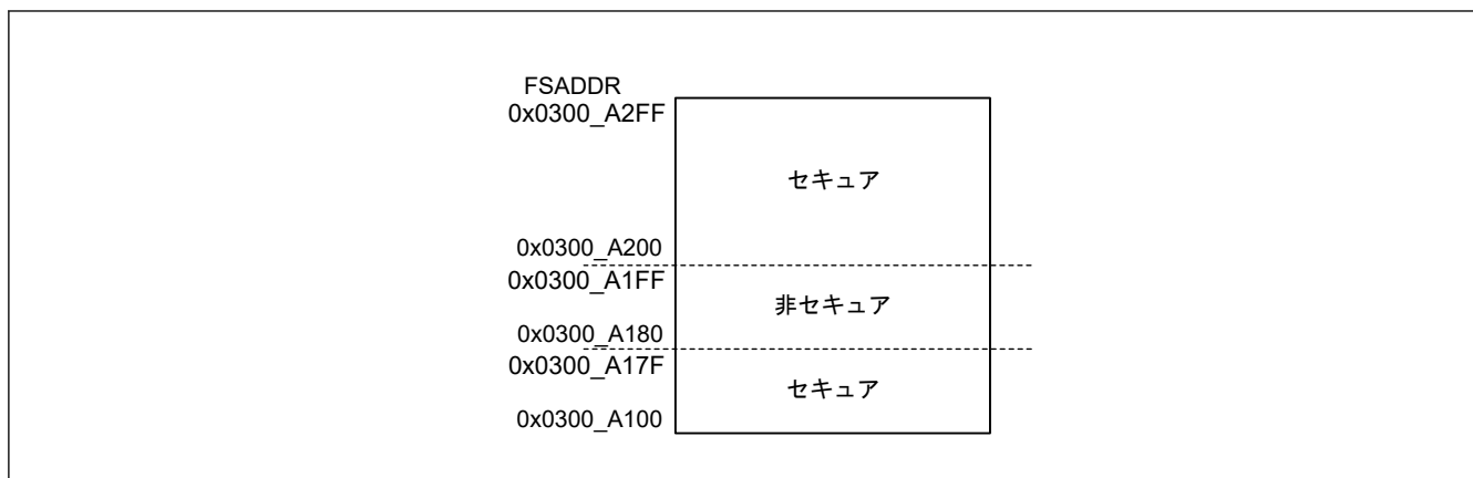
図 52.41 オプション設定メモリ内のセキュア領域と非セキュア領域（セキュアエイリアスの場合）
