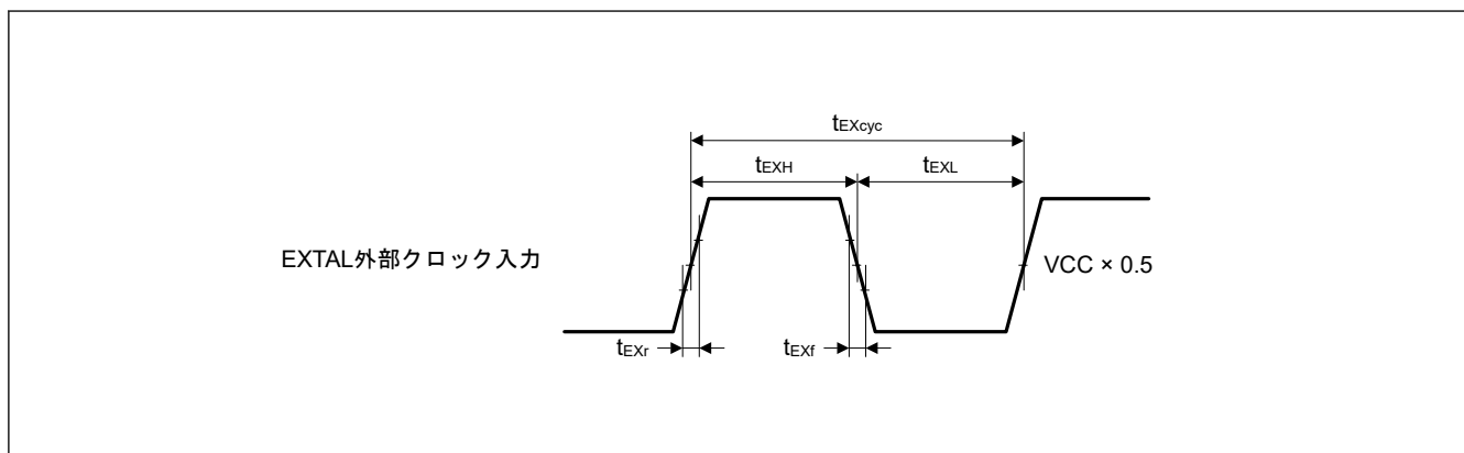
図 60.16 EXTAL 外部クロック入力タイミング
