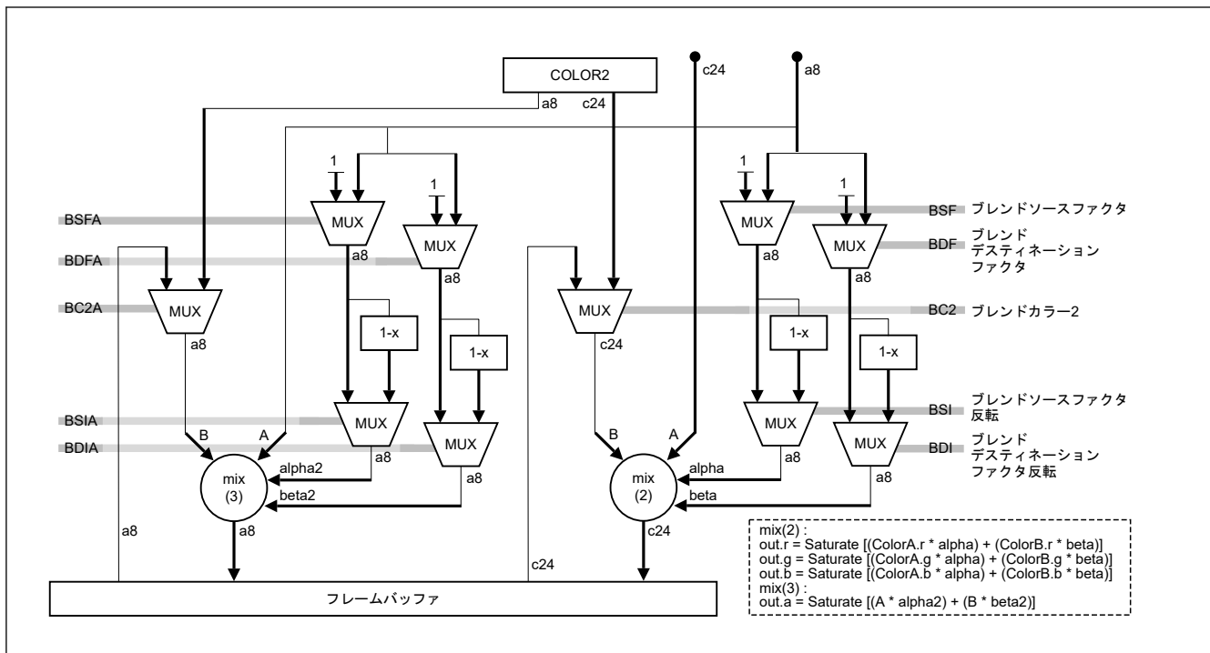
図 55.24 CONTROL2.USEACB = 1 の場合のアルファチャンネルおよびカラーチャンネルのブレンドユニット
