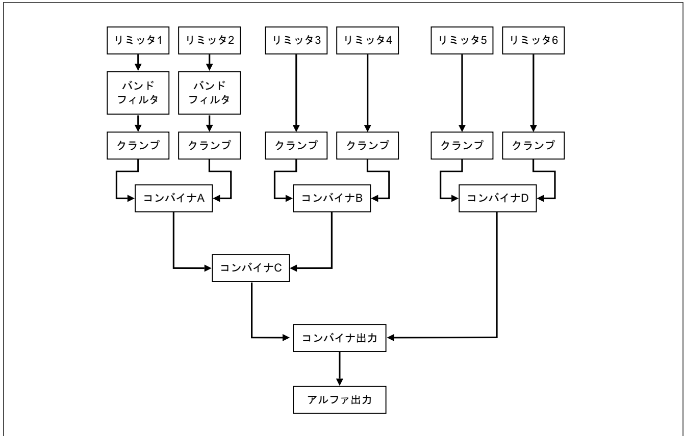
図 55.6 ラスタライゼーションユニットのブロック図
