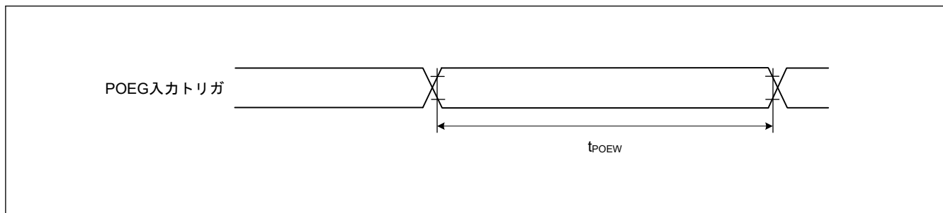
図 60.44 POEG 入力トリガタイミング
