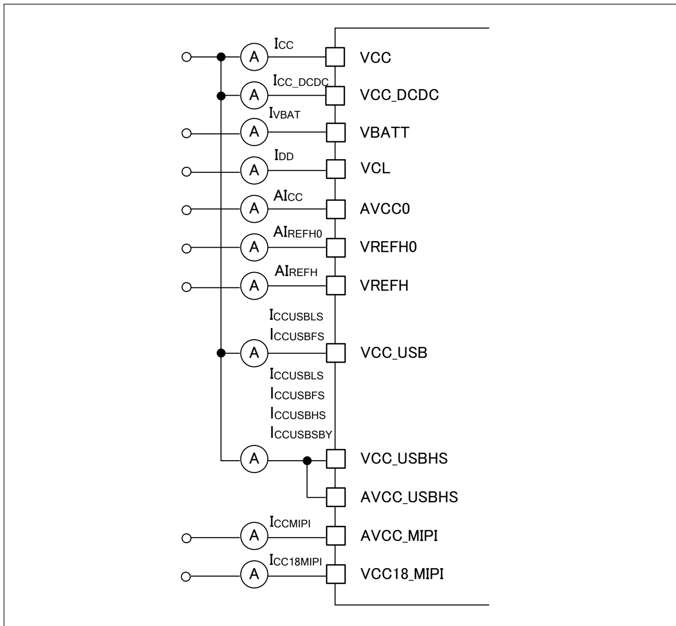
図 60.2 消費電流測定図
