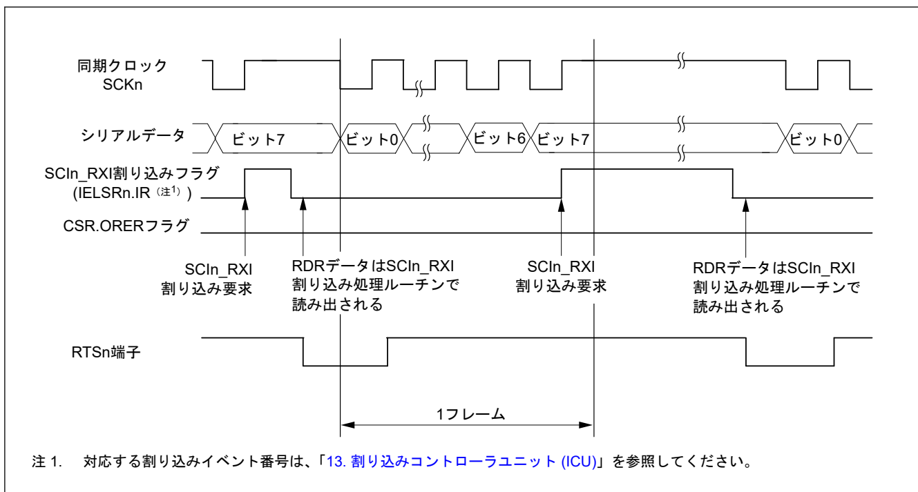
図 31.68 クロック同期式モードにおけるシリアル受信の動作例 (2) (RTS 機能を使用する場合)
