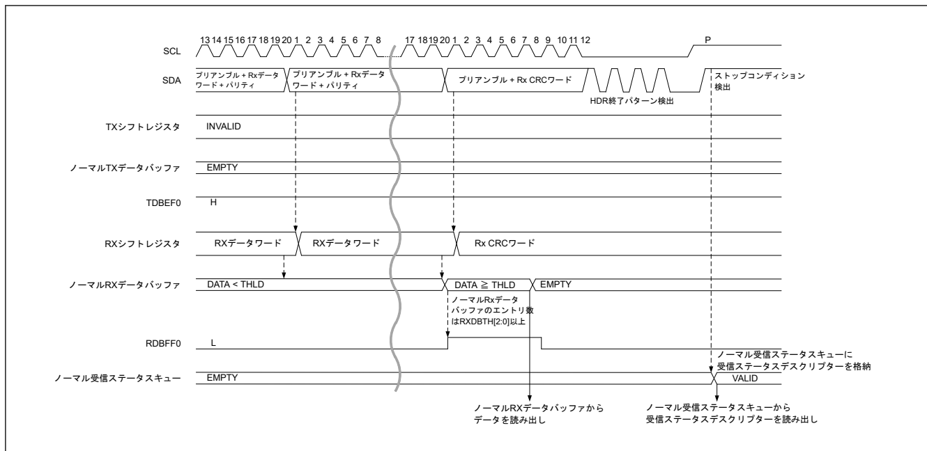
図 33.55 HDR データ書き込み転送 (HDR-DDR) タイミング (3/3)
