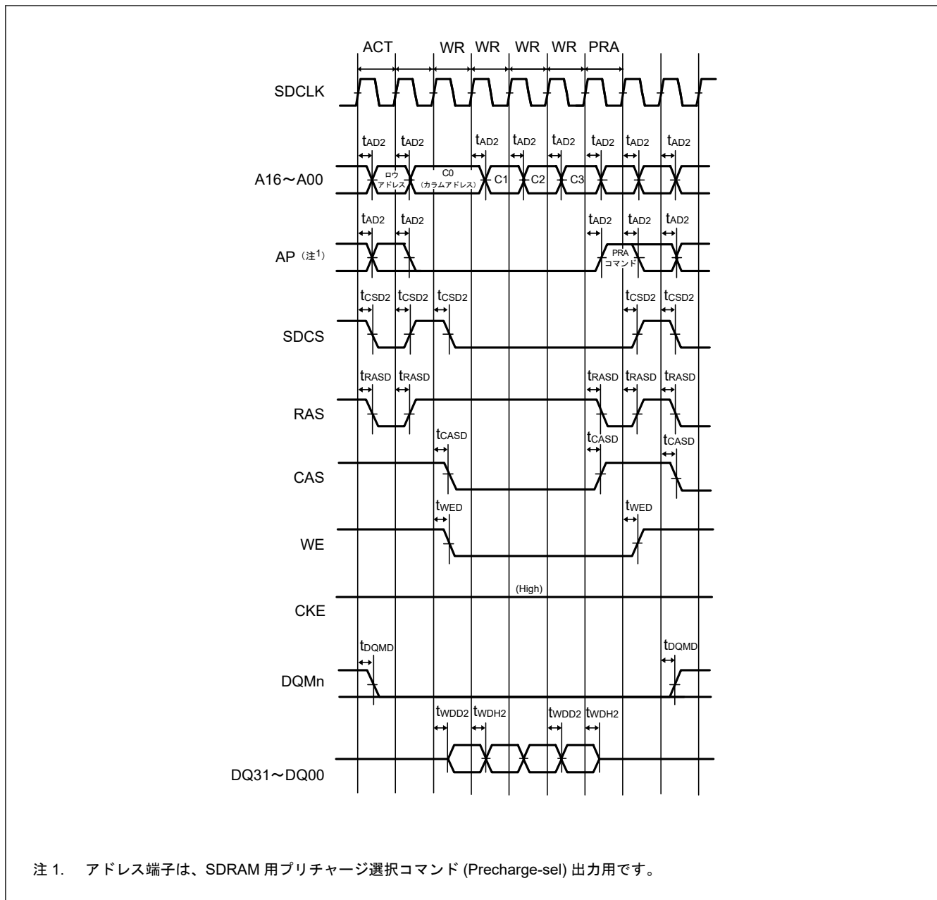
図 60.38 SDRAM マルチライトのタイミング
