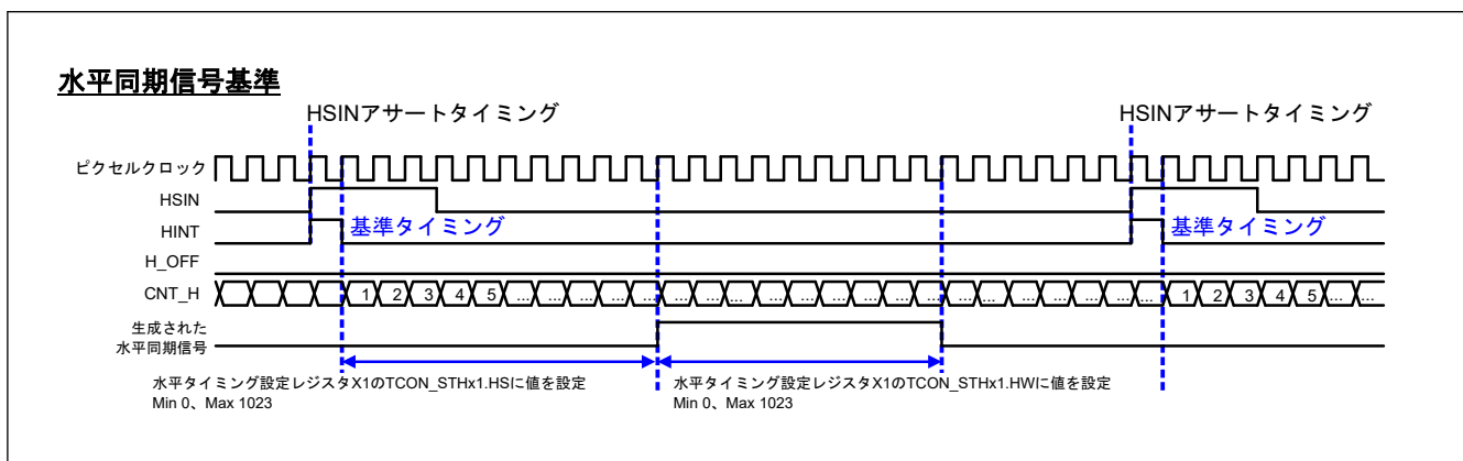
図 56.20 入力水平同期信号 (HSIN) に基づく信号生成
