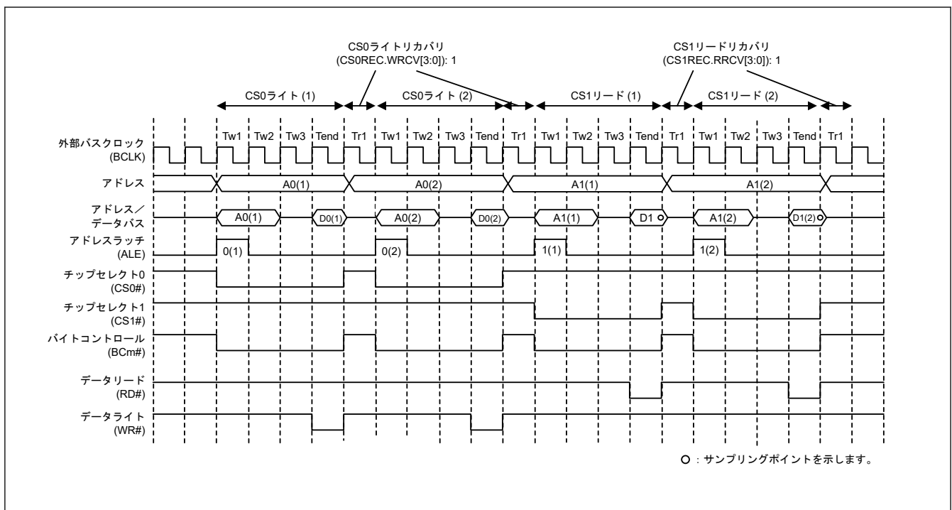
図 14.34 バスアクセスが分割された場合のリカバリサイクルの動作例（アドレス／データマルチプレクス I/O インタフェースの場合）(m = 0, 1)
