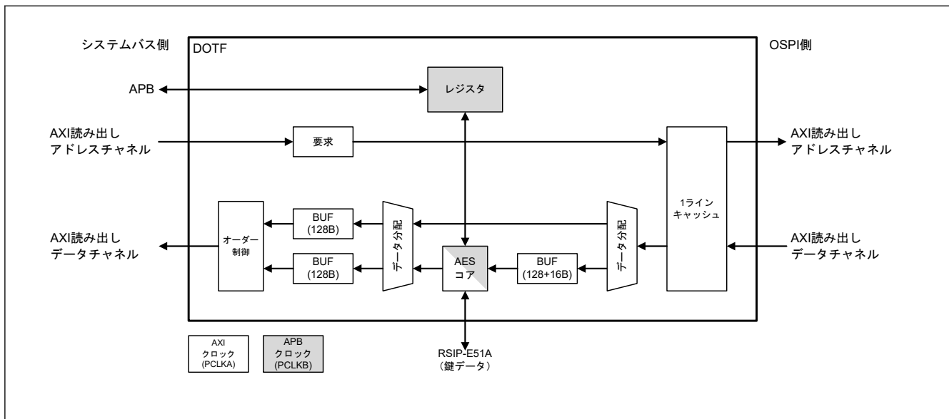
図 38.1 ブロック図
