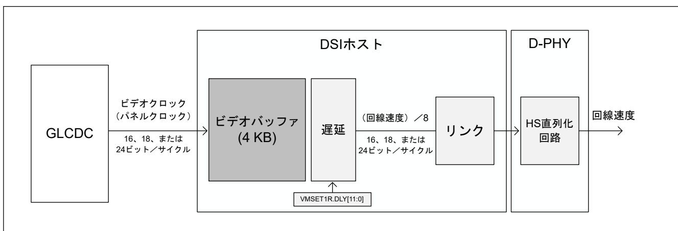
図 58.5 ビデオバッファと遅延制御
