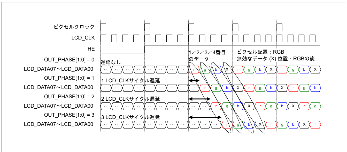
図 56.5 シリアル RGB888 (4 倍速) 出力タイミング
