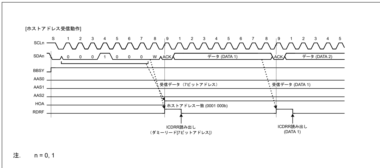
図 32.29 ホストアドレス受信時に HOA フラグが 1 になるタイミング
