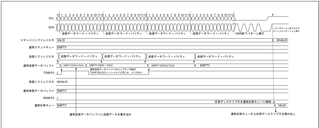
図 33.29 HDR データ書き込み転送 (HDR-TSP、TSL) タイミング (2/2)
