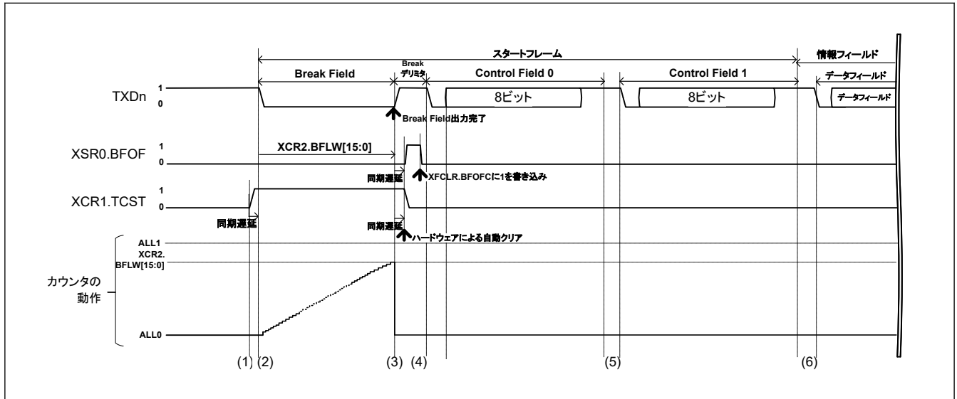
図 31.102 スタートフレーム送信例
