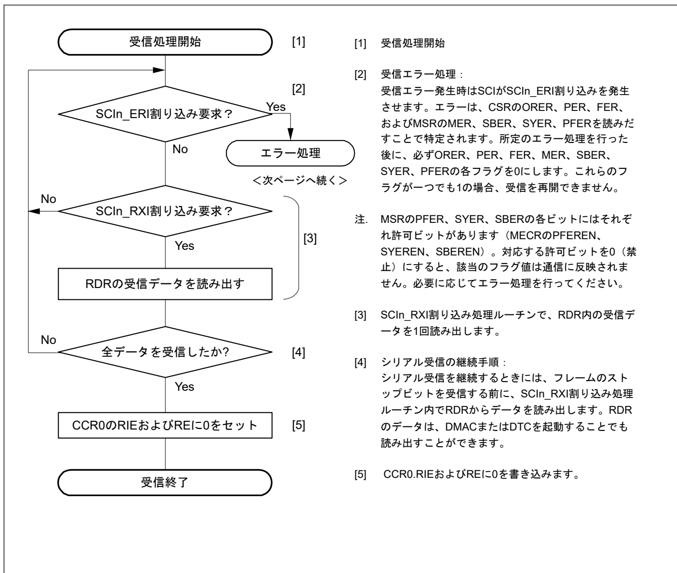
図 31.57 マンチェスタモードにおけるシリアルデータ受信フローチャートの例（正常受信）
