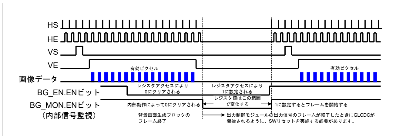
図 56.25 通常動作時の停止と再開
