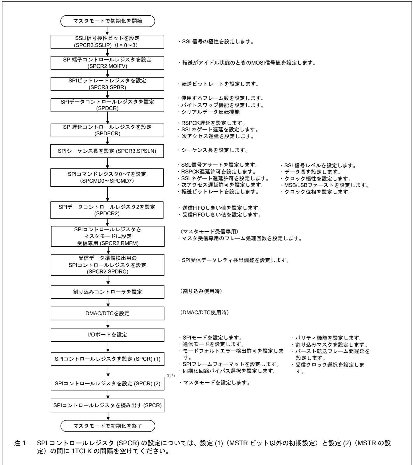
図 36.63 マスタモード時の SPI 動作の初期化フロー例
