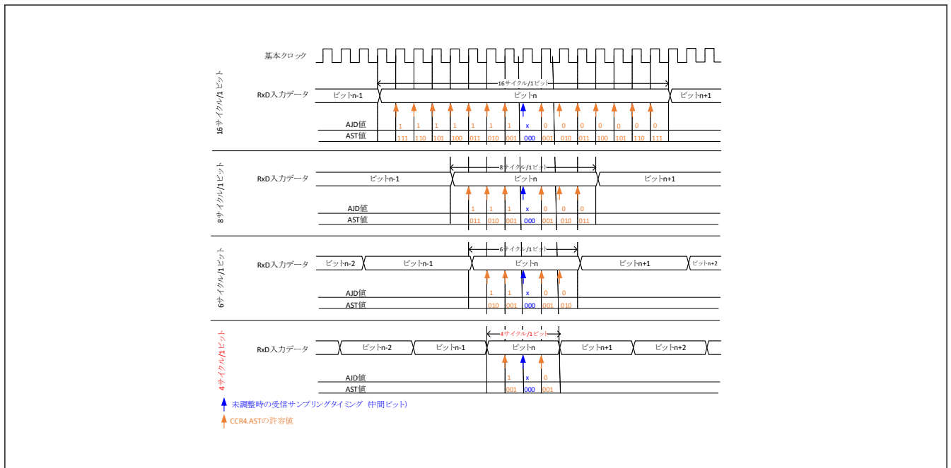
図 31.29 受信サンプリングタイミングの調整動作の概要 (内部クロックを使用した調歩同期式モード)
