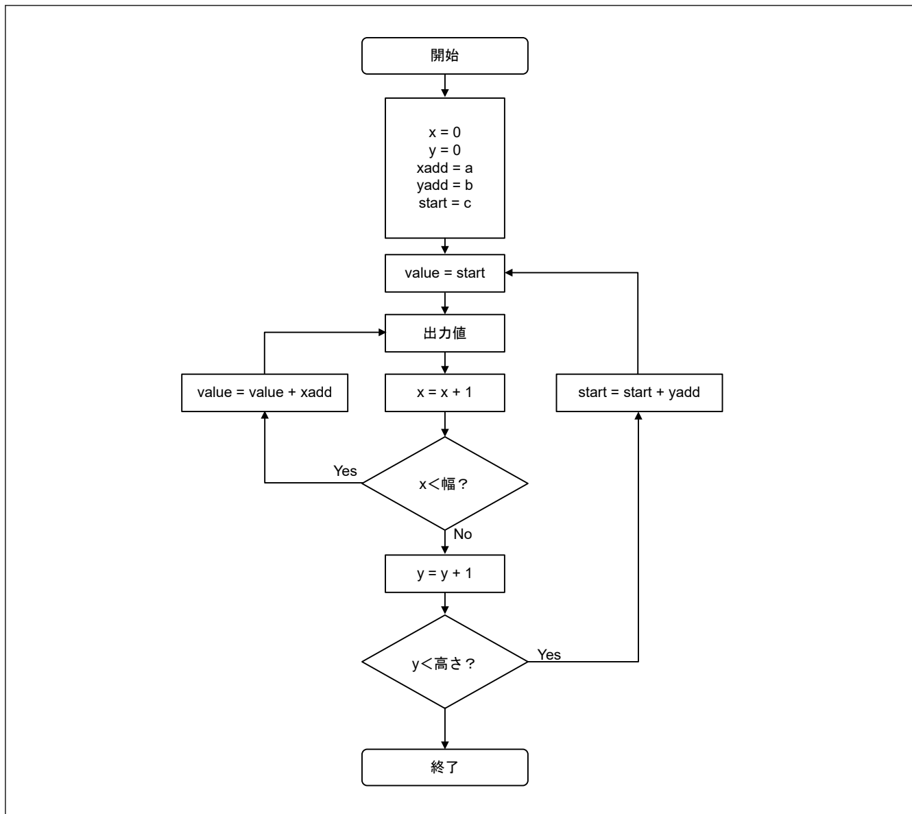
図 55.8 線形リミッタの動作フロー
