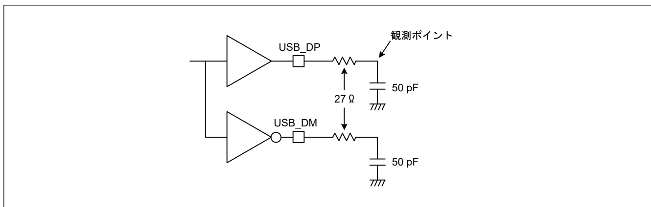
図 60.114 フルスピードモードにおける測定回路
