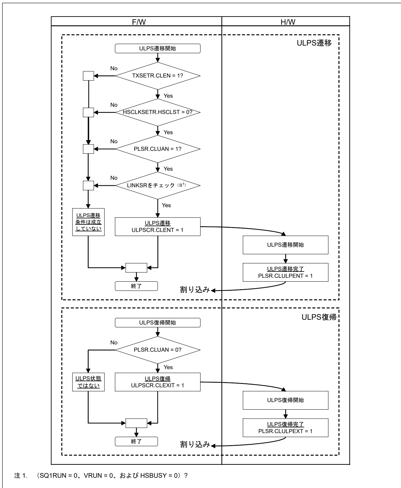
図 58.7 ULPS 遷移/復帰 (クロックレーン)
