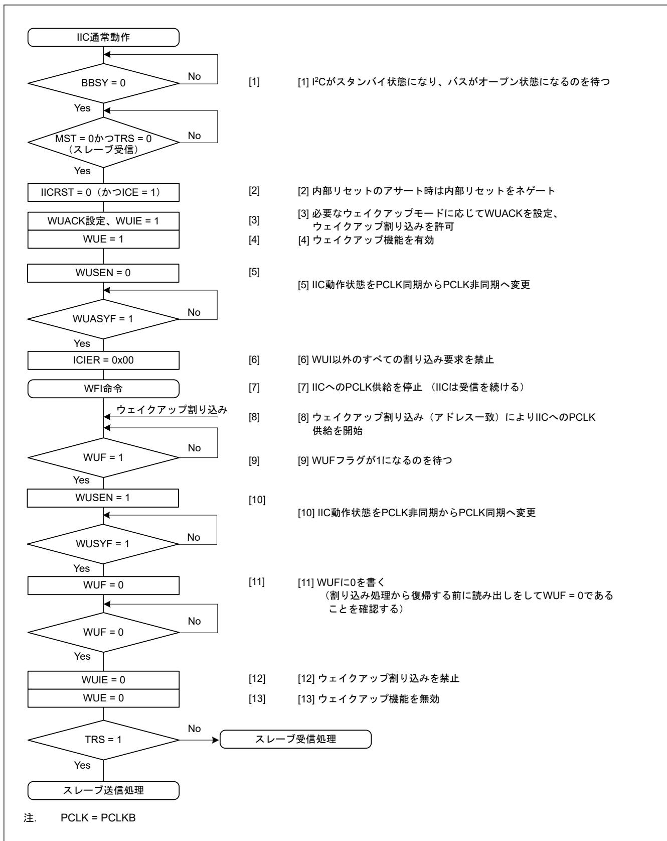
図 32.30 ノーマルウェイクアップモード1の動作例 (スレーブアドレス一致時のウェイクアップ割り込みによるウェイクアップの場合)
