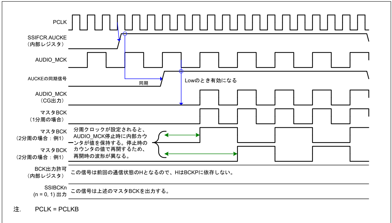
図 39.27 通信停止からマスターモード通信開始までの動作のタイミング図
