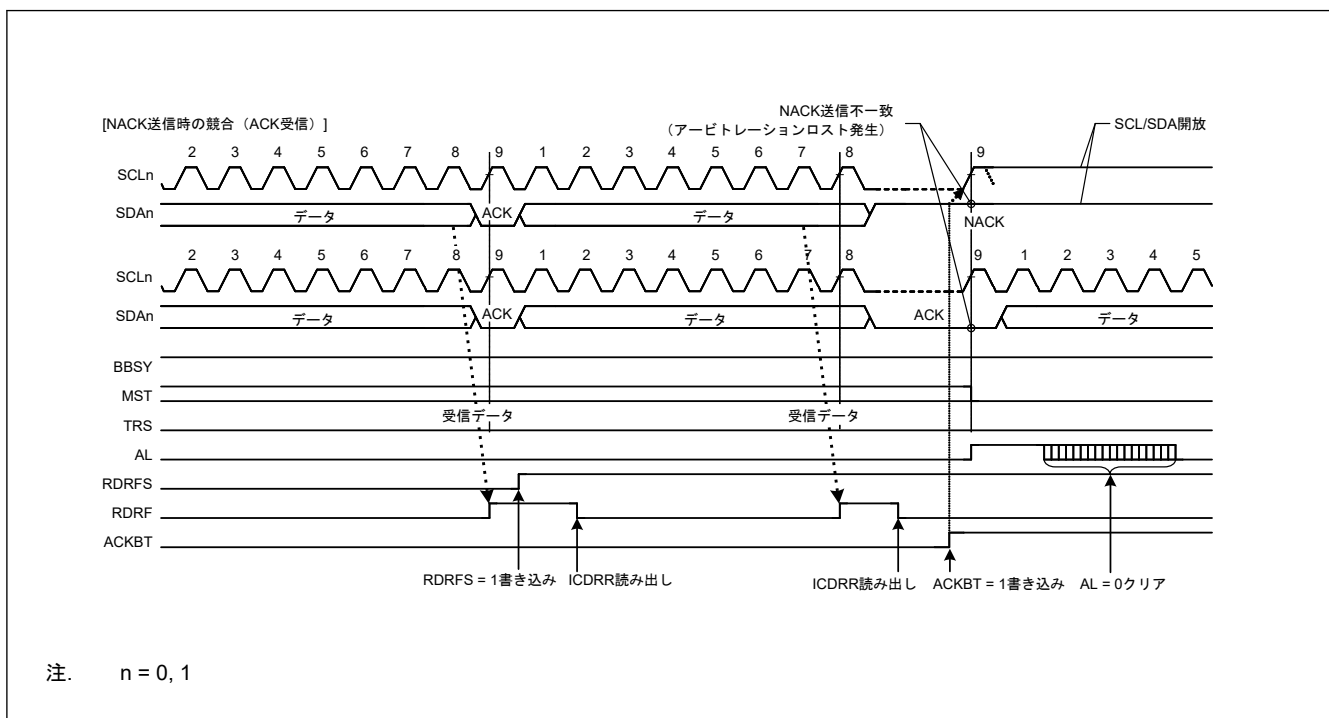
図 32.43 NACK 送信中のアービトレーションロスト検出の動作例 (NALE = 1 の場合)
