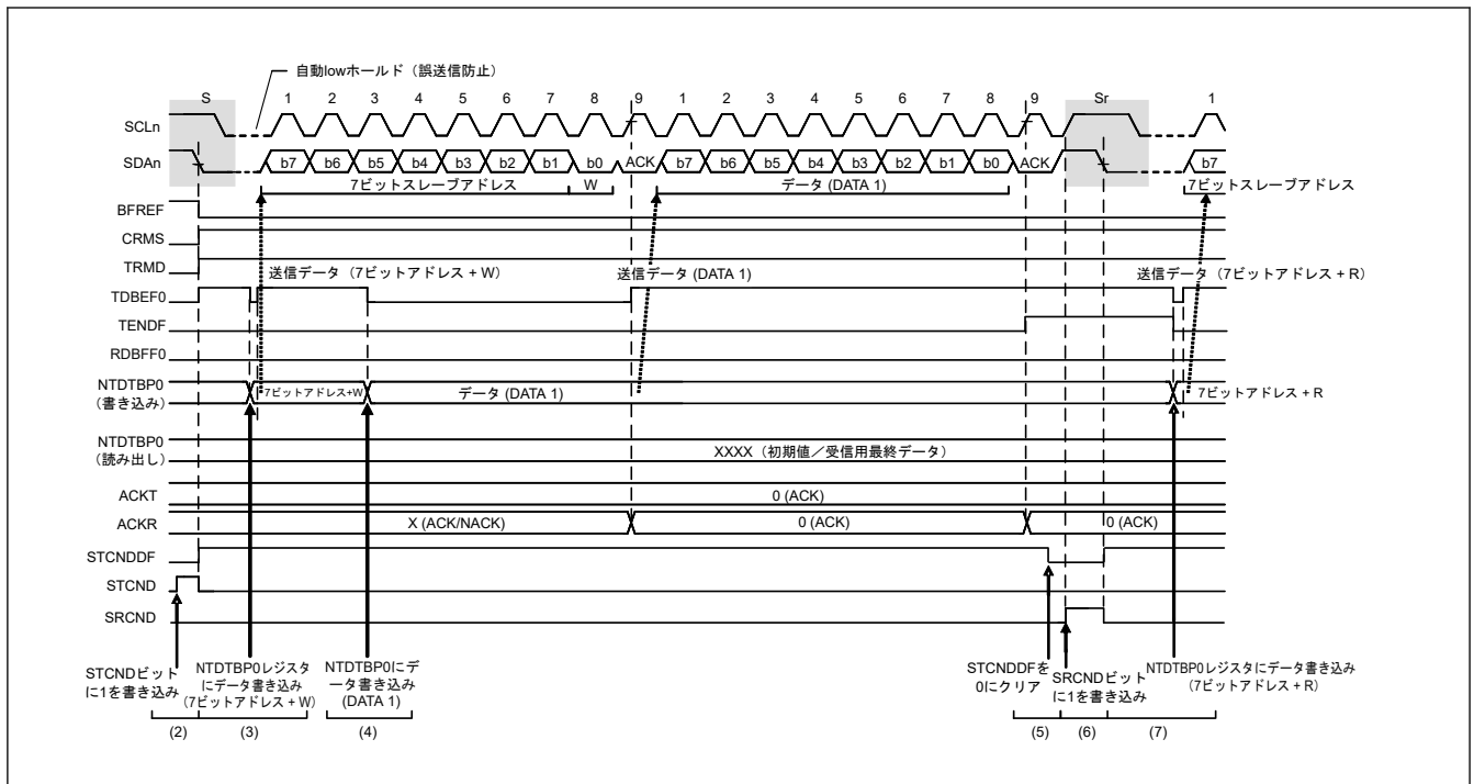
図 33.80 マスタ送信後の繰り返しのスタートコンディション発行タイミング
