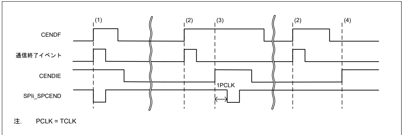
図 36.46 通信終了割り込みの動作例 (イネーブル制御)
