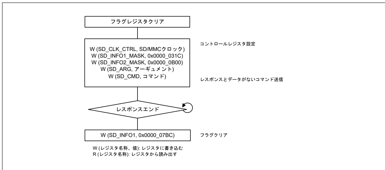
図 40.9 レスポンスまたはデータがないコマンドのフロー例
