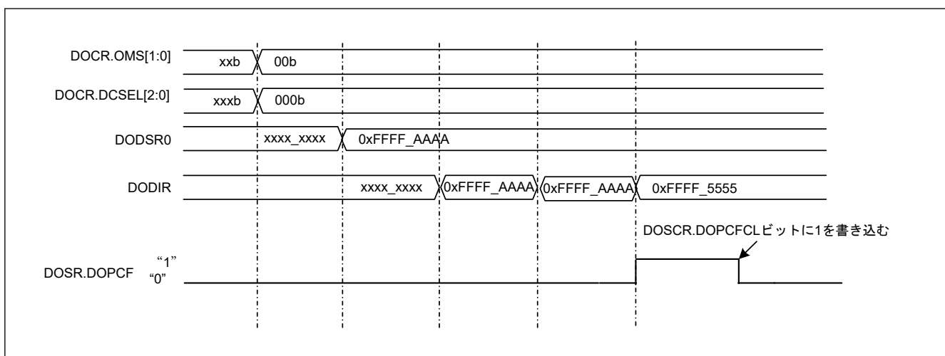
図 49.2 データ比較モードの動作例 (検出条件 : 不一致)
