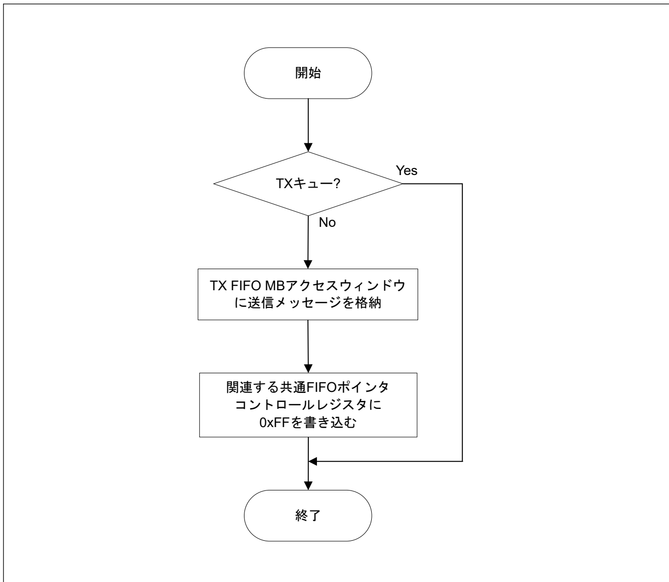
図 34.45 TX FIFO の送信要求手順
