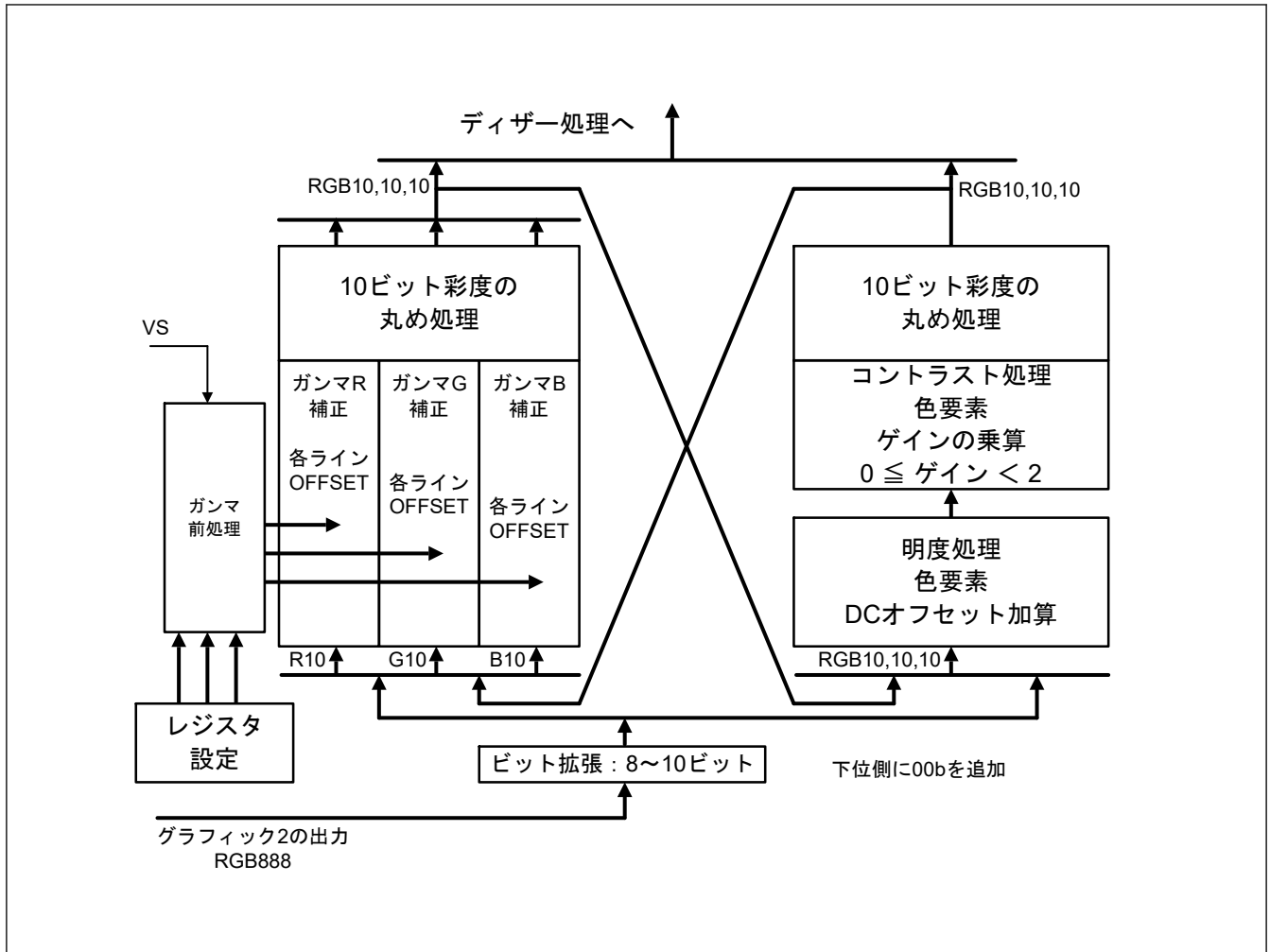
図 56.6 パネル指向補正回路の構成
