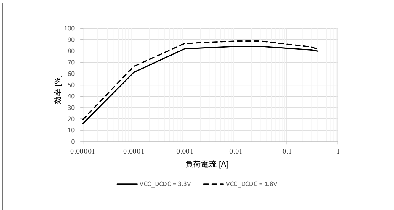
図 60.11 Low-speed モードおよびソフトウェアスタンバイモード、 T_j = 25\text{ }^\circ\text{C} における標準 DCDC 効率 (%) と負荷電流 (A)
