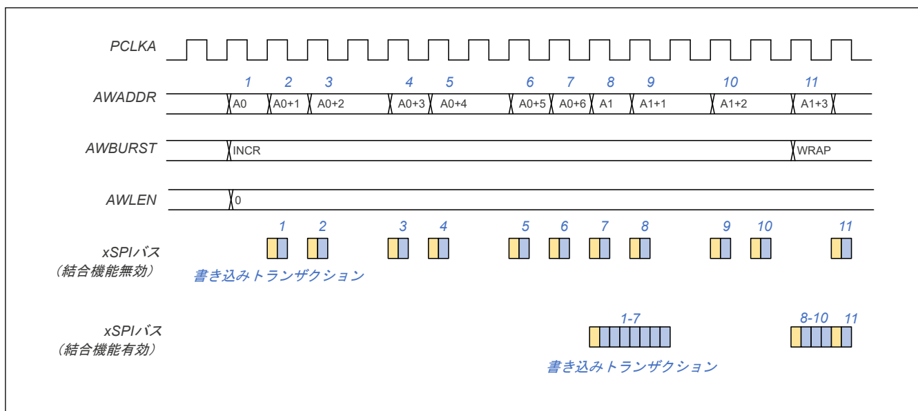
図 37.14 結合機能
