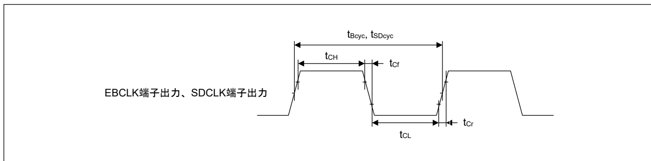
図 60.15 EBCLK および SDCLK の出力タイミング
