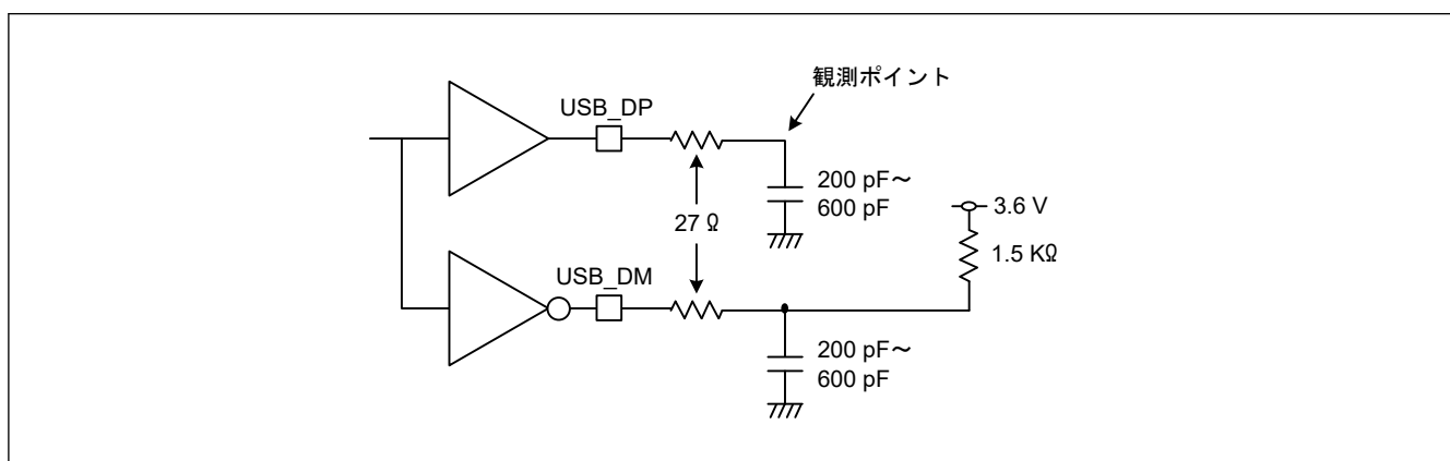
図 60.112 Low-speed モードにおける測定回路
