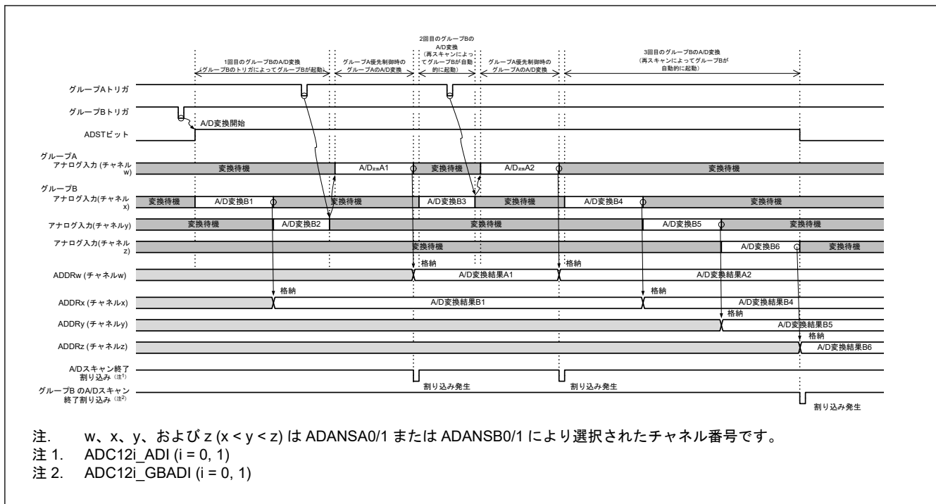
図 45.28 グループ優先動作の例 1-2 : グループ B 再スキャン中のグループ A トリガ入力、再スキャンあり (ADGSPCR.GBRSCN = 1, ADGSPCR.GBRP = 0、および ADGSPCR.LGRRS = 0 の場合)
