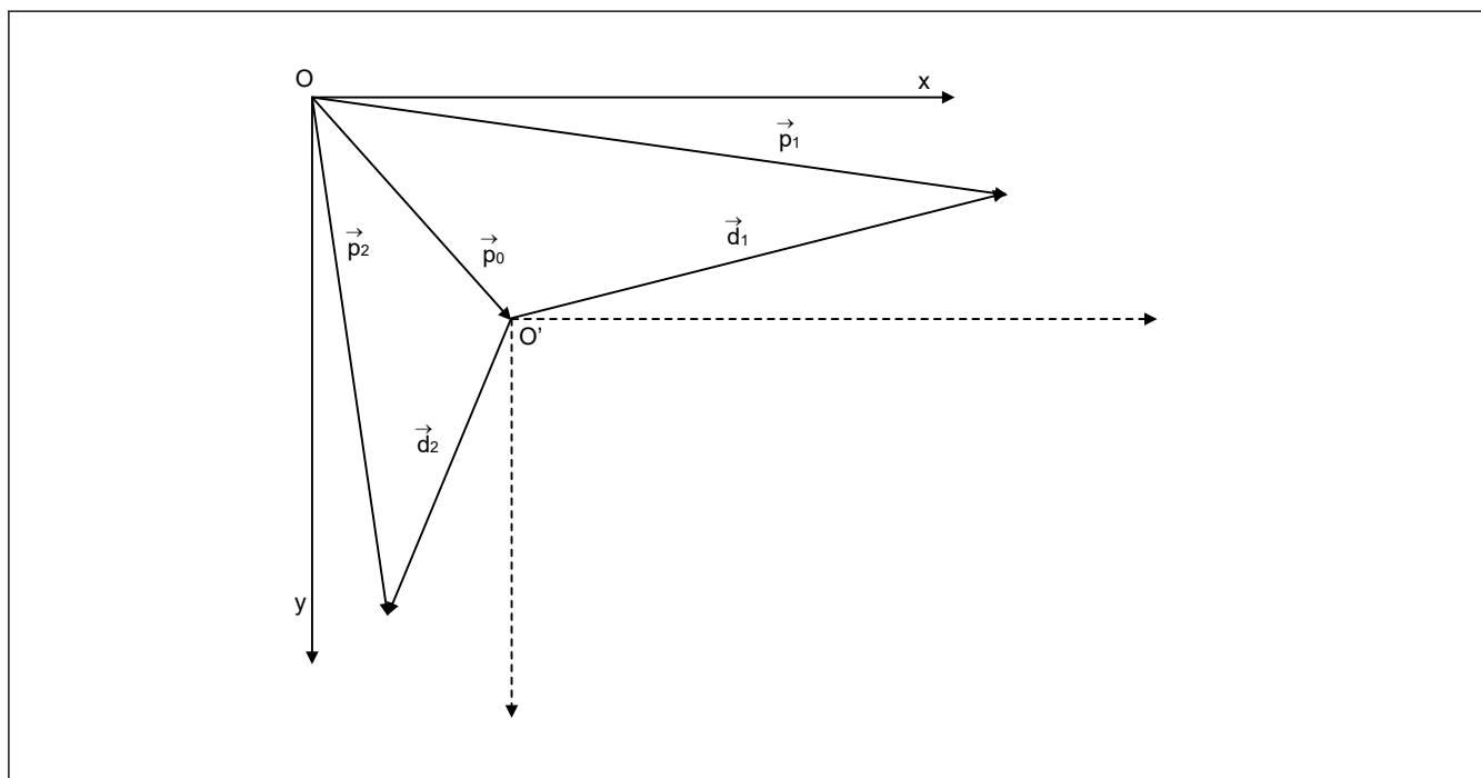
図 55.20 テクスチャマッピング、オブジェクト空間、計算を簡素化するための座標系 O から O' への変換
