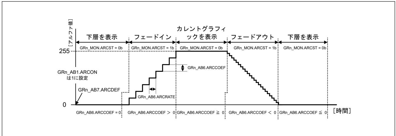
図 56.9 アルファブレンド値の更新
