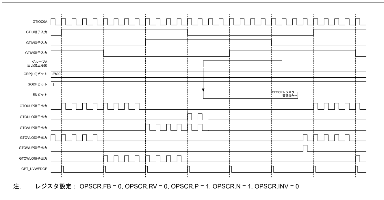
図 21.67 グループ出力禁止制御動作例
