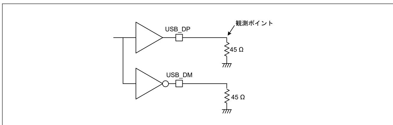
図 60.118 High-speed モードにおける測定回路
