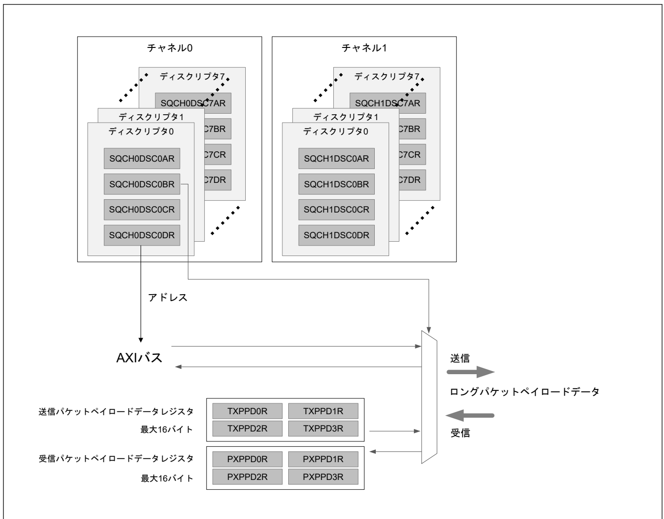
図 58.4 シーケンス動作のためのディスクリプタとパケットデータバッファ
