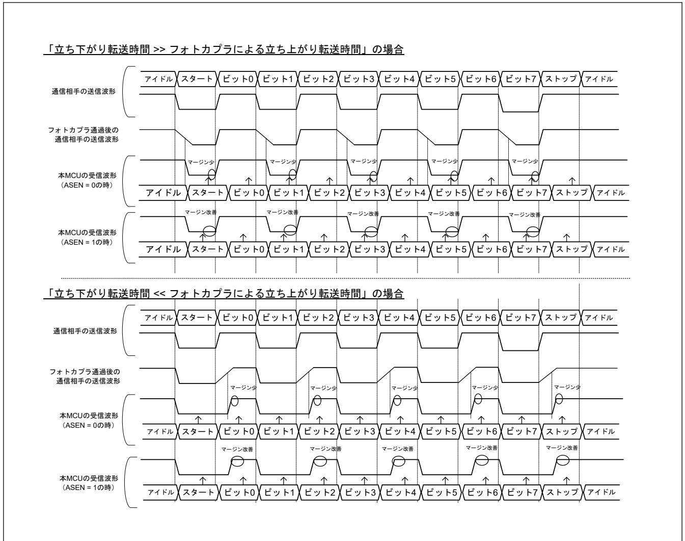
図 31.28 受信サンプリングタイミング調整機能による受信マージン向上の例
