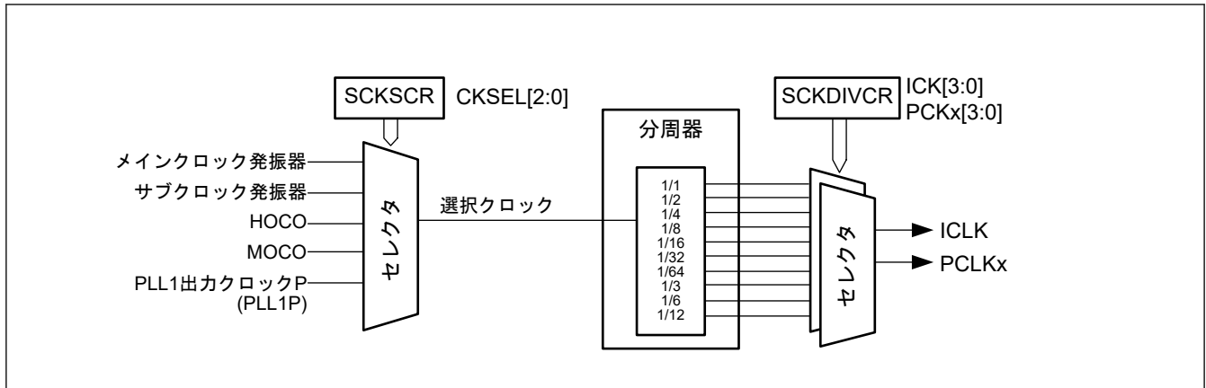
図 8.11 クロックソースセレクタのブロック図
