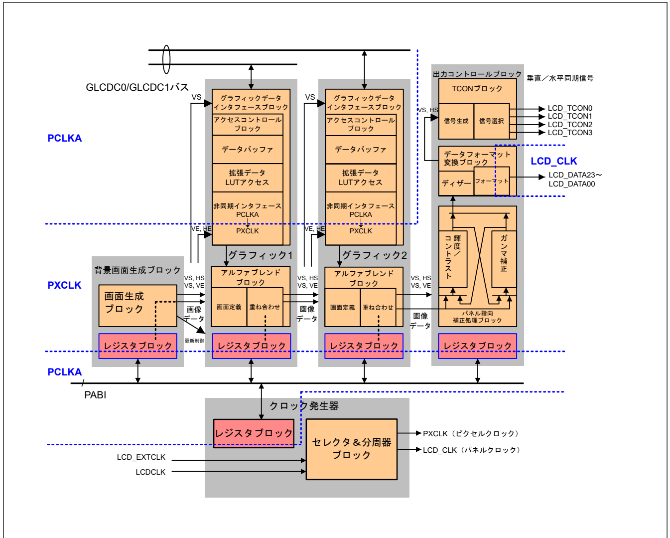
図 56.2 GLCDC の構成
