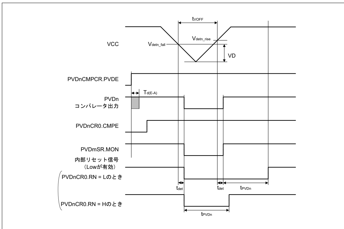
図 60.123 電圧検出回路タイミング ( V_{detn} ) ( n = 1, 2 )
