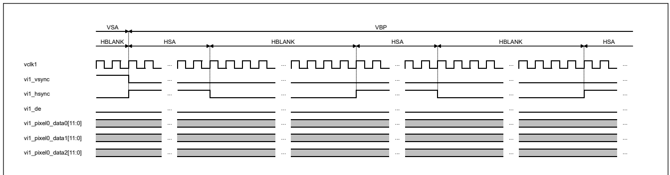
図 58.11 VSA 終了と VBP 開始
