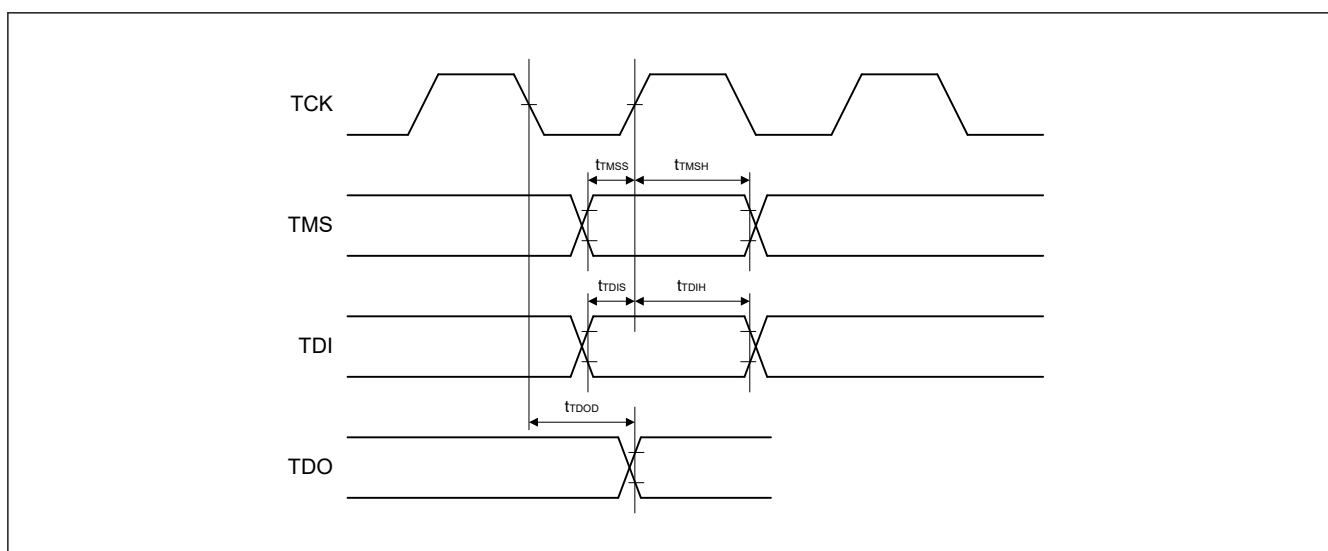
図 60.128 バウンダリスキャン入出力タイミング (1)
