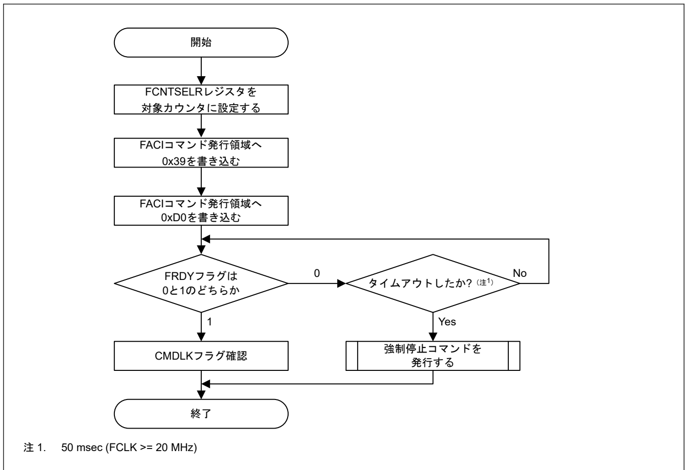
図 52.28 カウンタ読み出しコマンドの使用法
