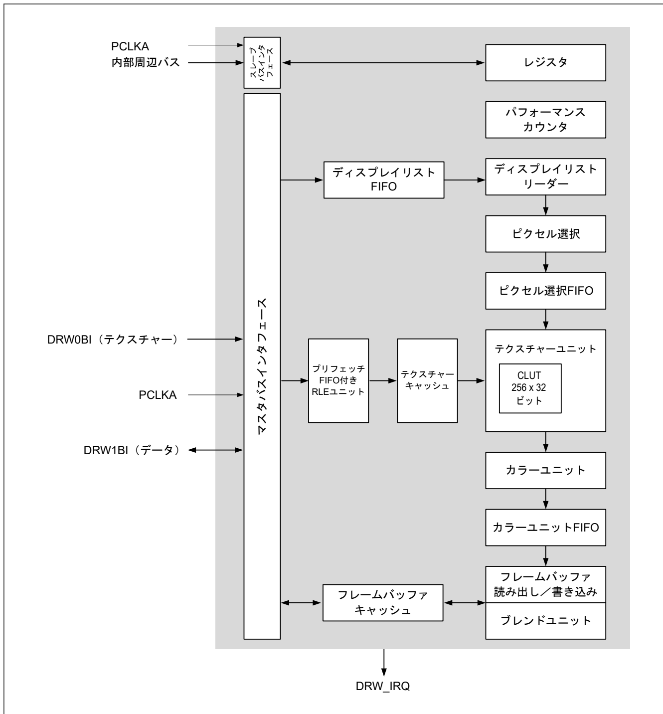
図 55.3 2D 描画エンジンのブロック図
