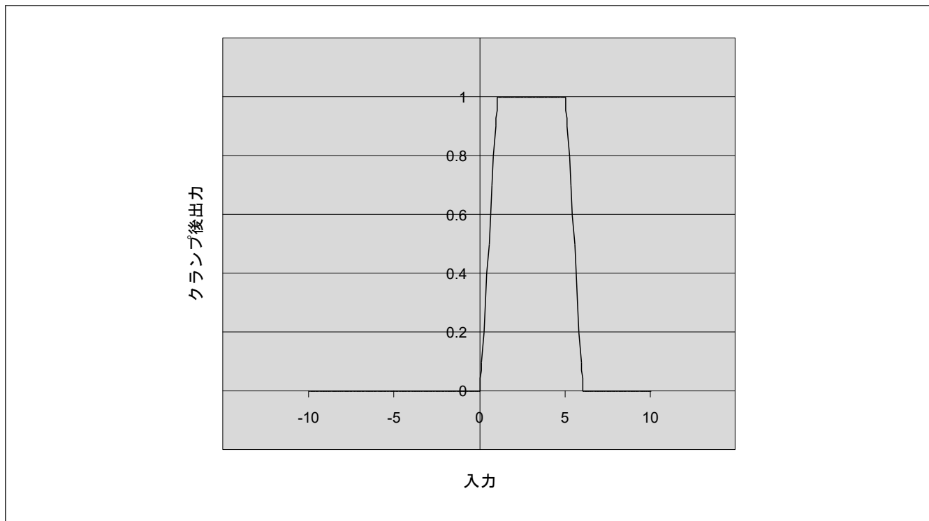
図 55.11 クランプ後のバンドフィルタ出力 (w = 7)
