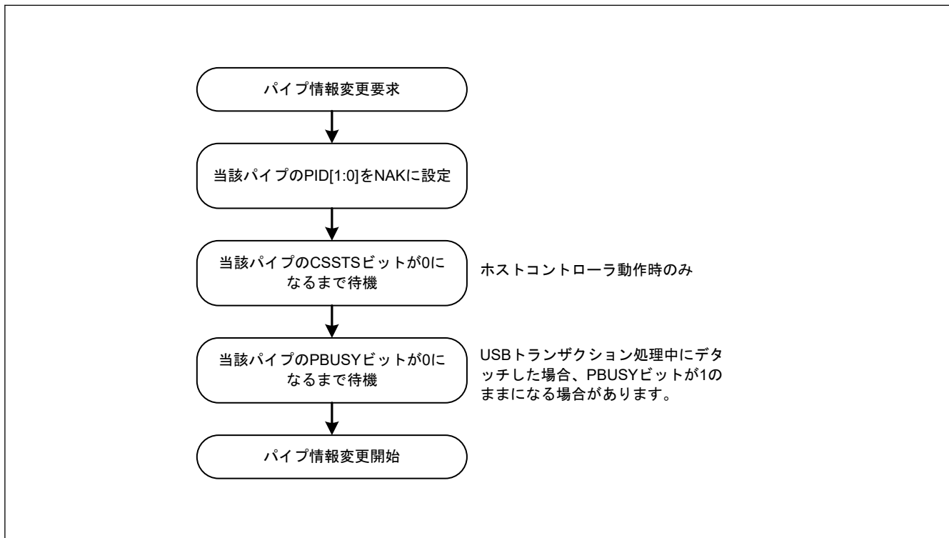
図 30.10 USB 通信が許可状態で PID[1:0]ビットが 01b (BUF 応答) のときのパイプ情報変更手順
