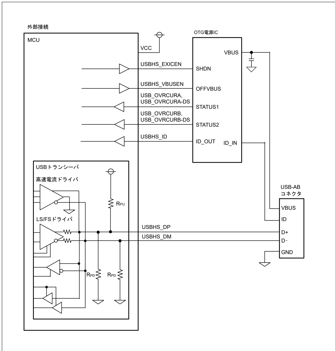
図 30.27 セルフパワードシステムでの OTG 接続例
