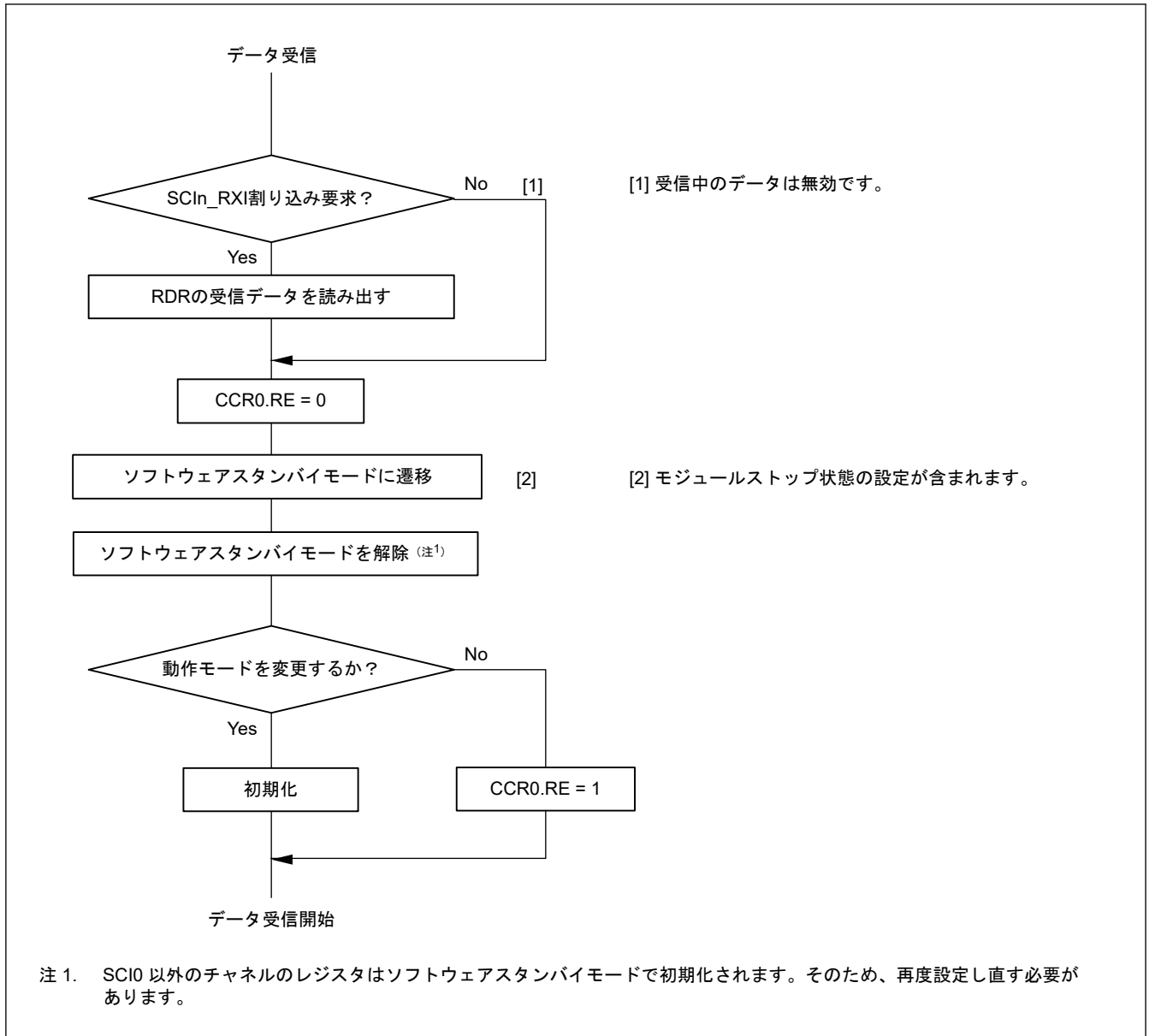
図 31.120 受信時にソフトウェアスタンバイモードへ遷移する場合のフローチャート例
