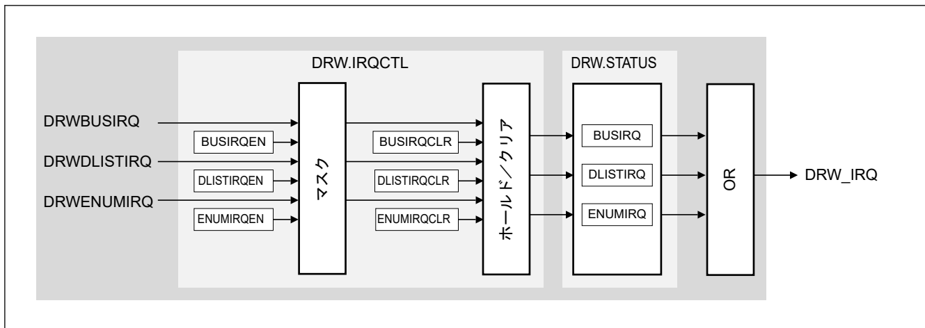
図 55.25 割り込みコントローラユニット (ICU)
