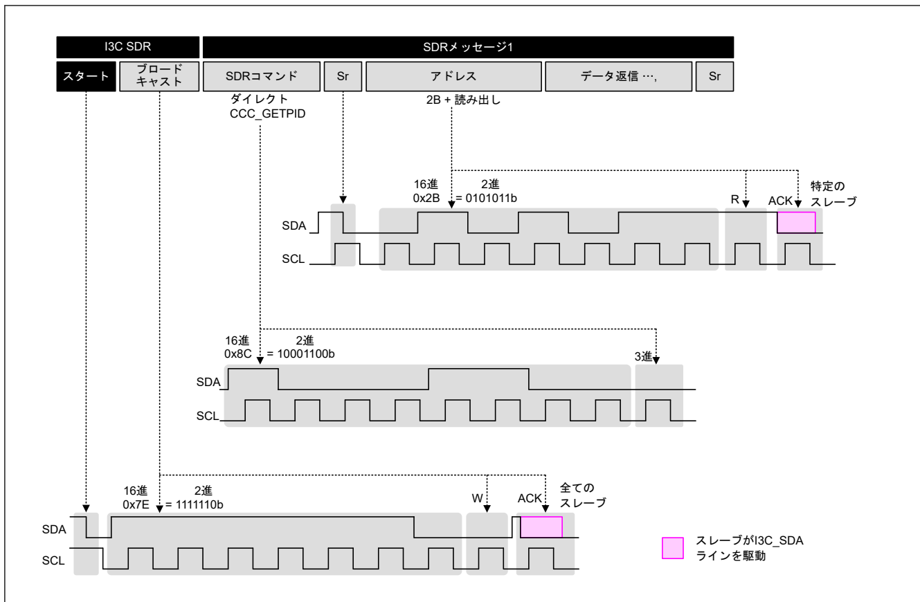
図 33.73 CCC ダイレクトアドレッシングを含む I3C SDR コーディングを使用した通信の例
