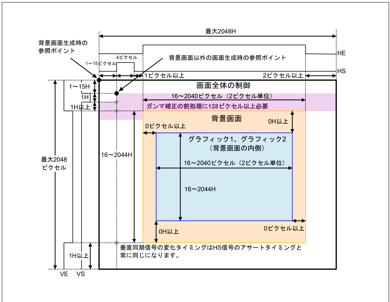
図 56.3 画面フォーマット
