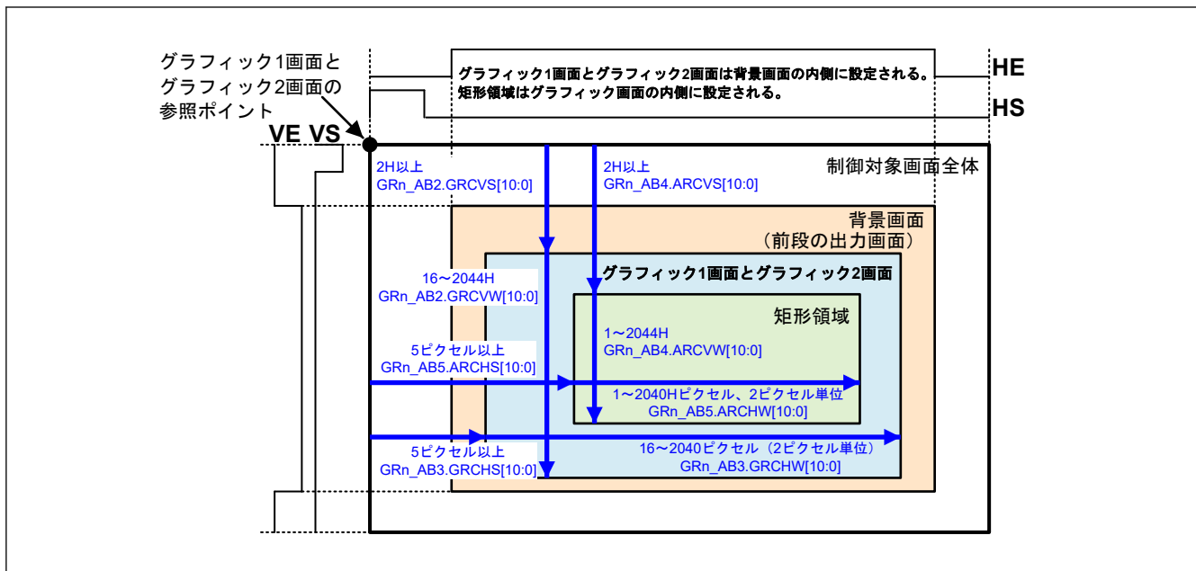
図 56.27 グラフィック 1 画面とグラフィック 2 画面の定義
