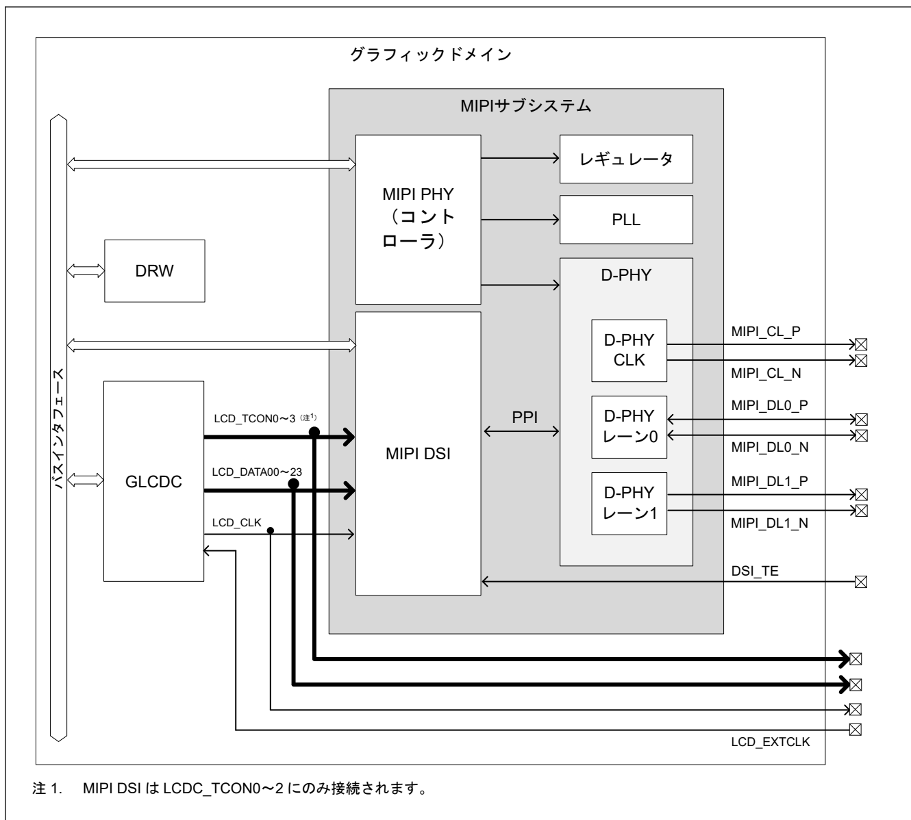
図 54.1 グラフィックドメインのブロック図
