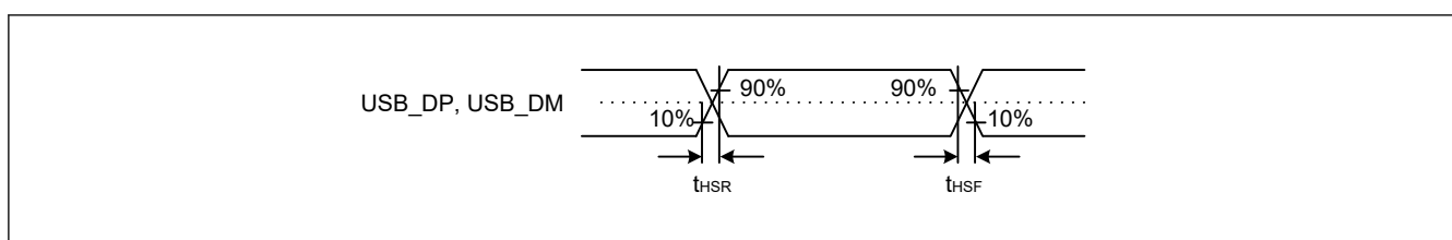
図 60.117 High-speed モードにおける USB_DP、USB_DM の出力タイミング
