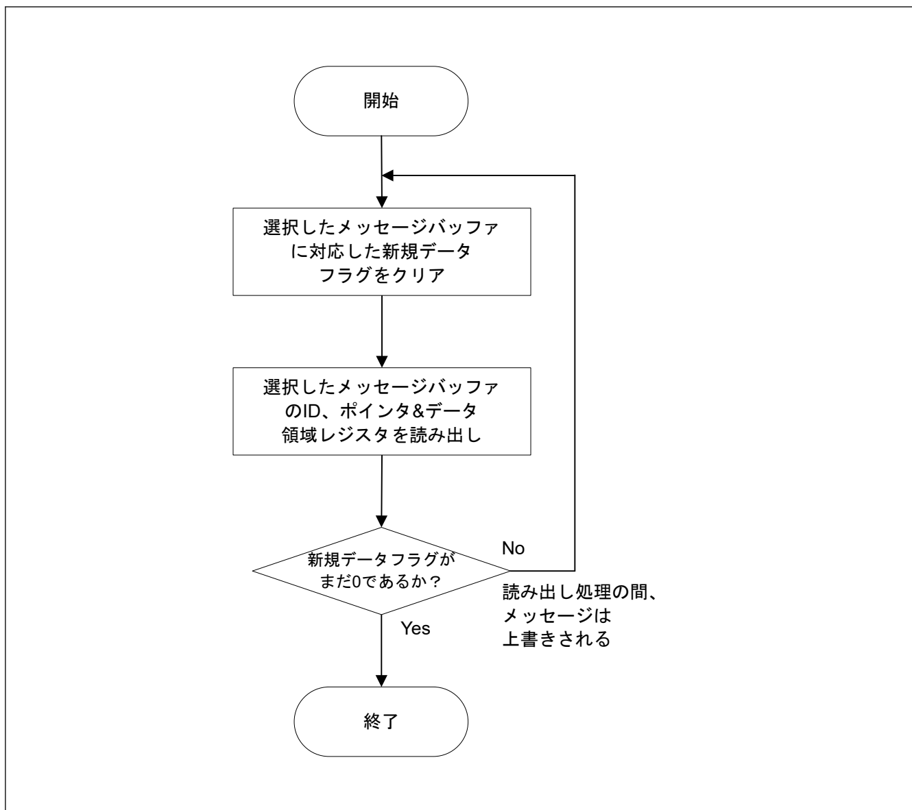
図 34.37 RX メッセージバッファの読み出し手順
