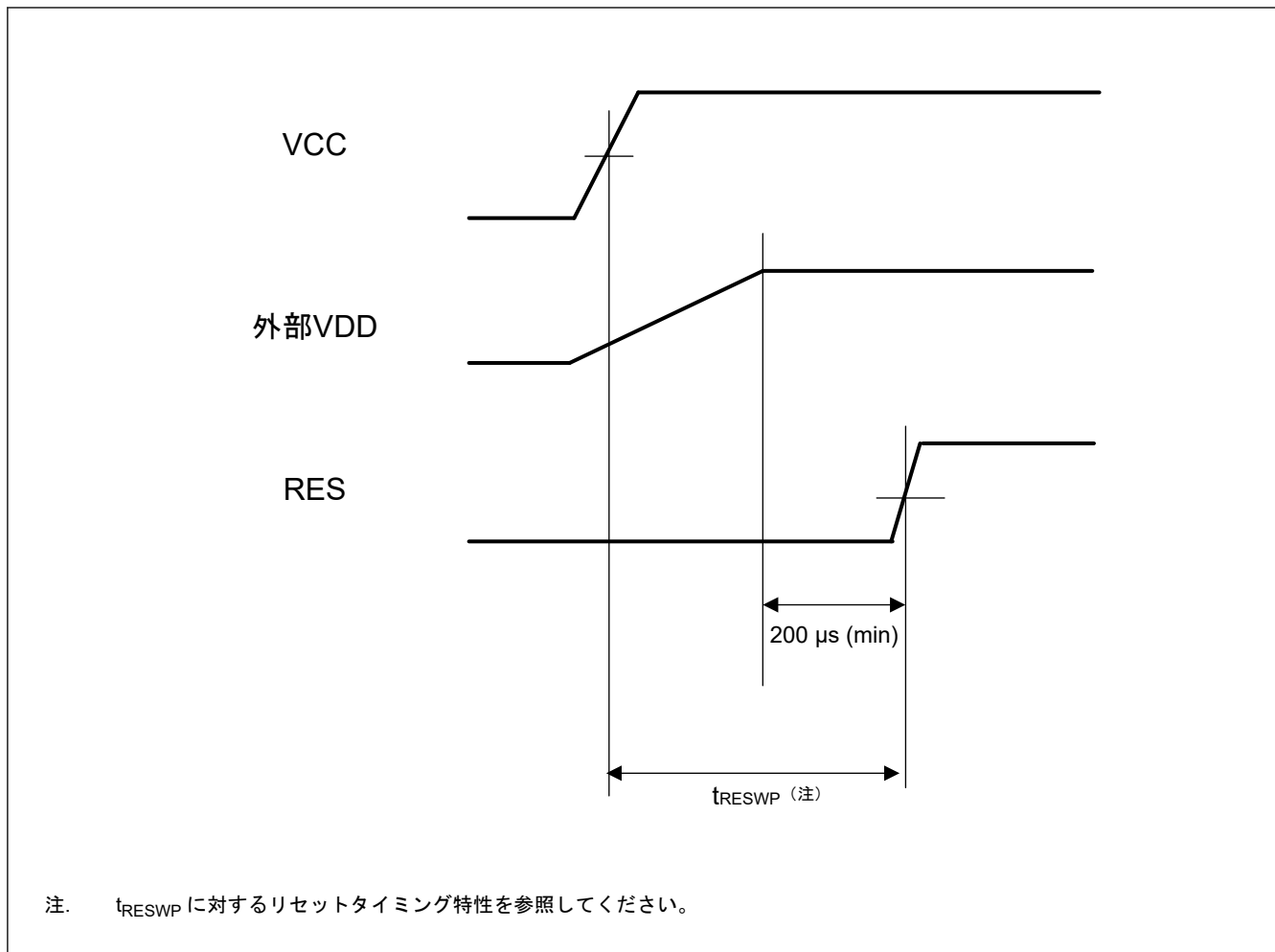
図 59.4 外部 VDD モードの電源起動シーケンス (RES 端子を使用する場合)
