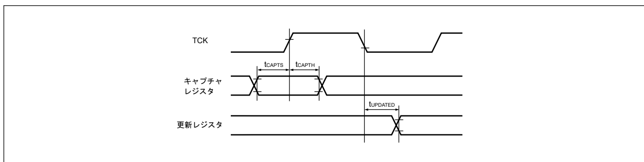
図 60.129 バウンダリスキャン入出力タイミング (2)
