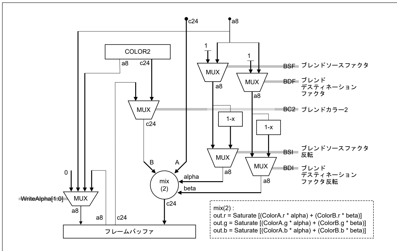
図 55.23 CONTROL2.USEACB = 0 の場合のカラーチャンネルブレンドユニット
