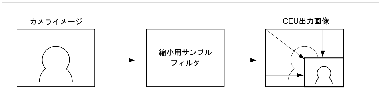
図 53.32 キャプチャ画像の縮小
