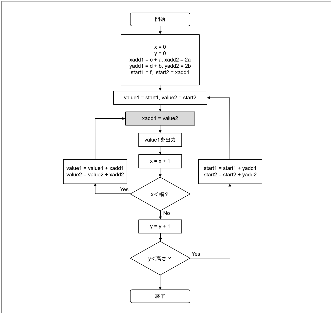
図 55.9 2 次リミッタの動作フロー
