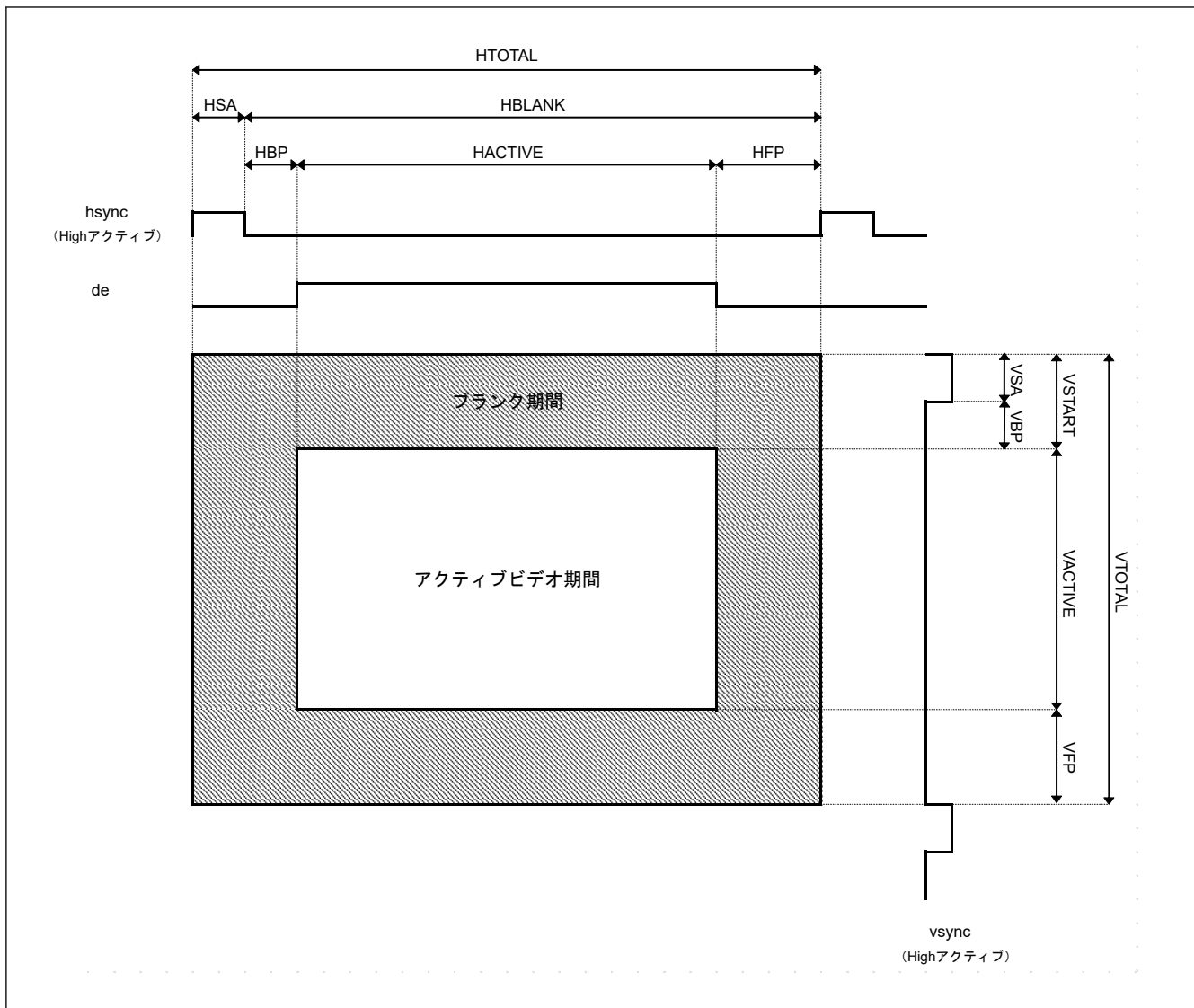
図 58.9 ビデオモードのタイミング
