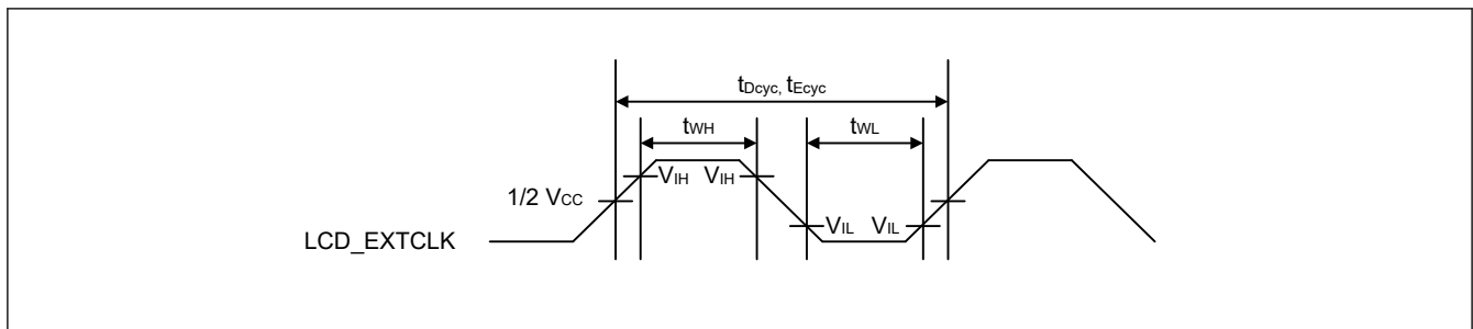
図 60.103 LCD_EXTCLK クロックタイミング
