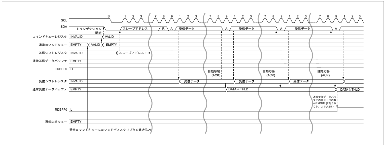
図 33.20 SDR データ読み出し転送タイミング (1/2)
