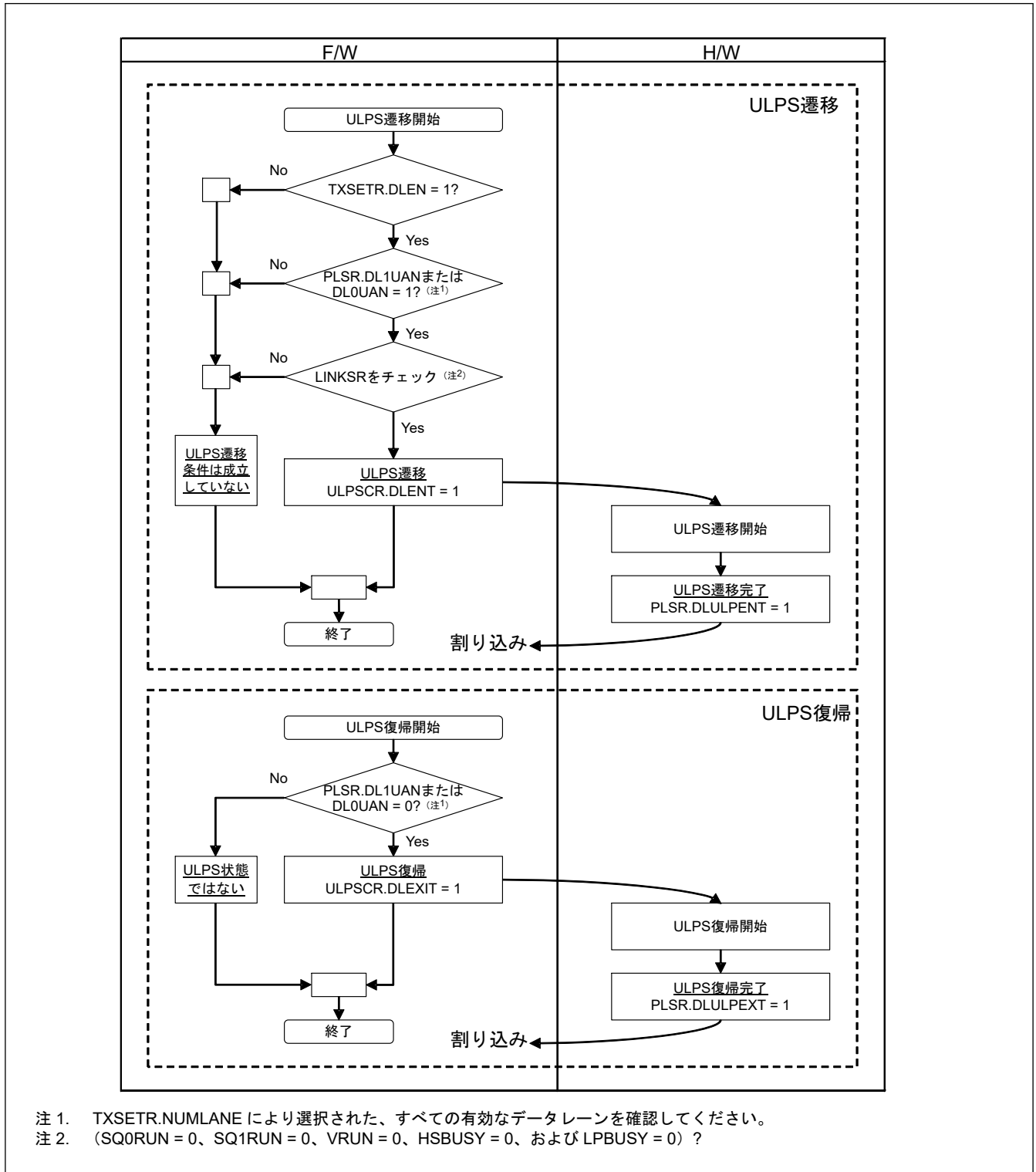
図 58.6 ULPS 遷移/復帰 (データレーン)
