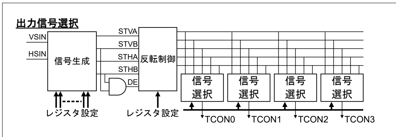
図 56.19 反転制御と出力信号選択の回路構成
