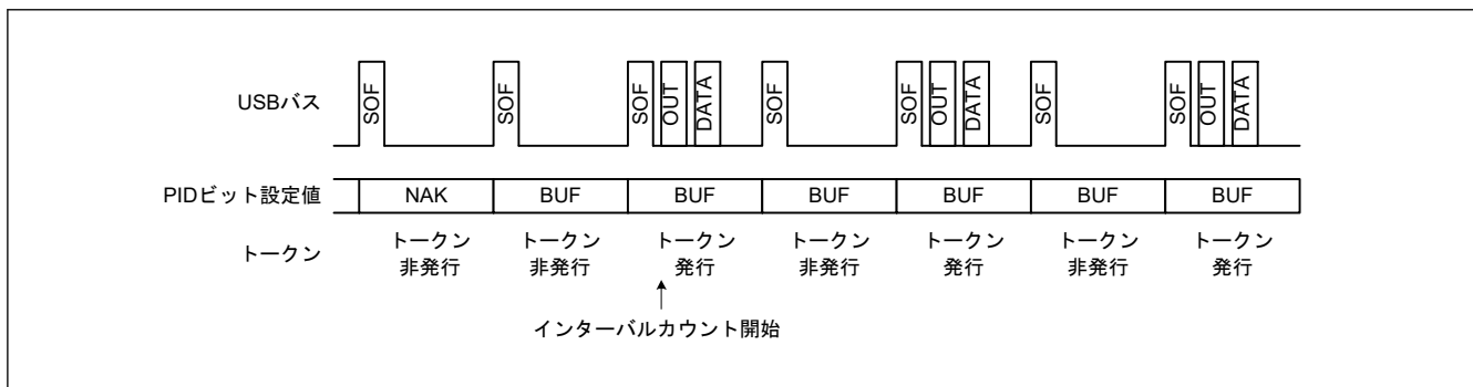
図 29.17 IITV = 1 の場合のトークン発行の有無
