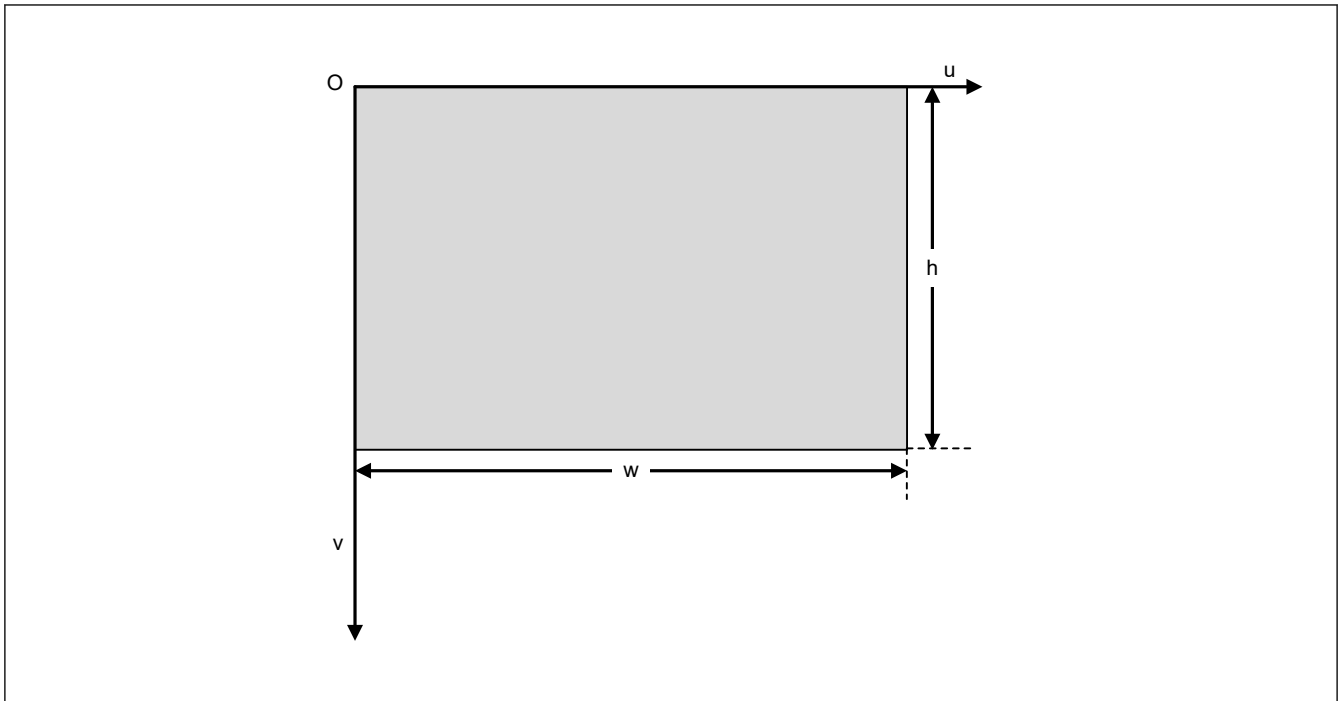
図 55.21 テクスチャマッピング、テクスチャ空間、幅 w 高さ h のテクスチャ
