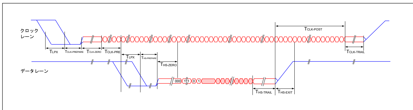
図 57.1 通常モードでの高速データ送信
