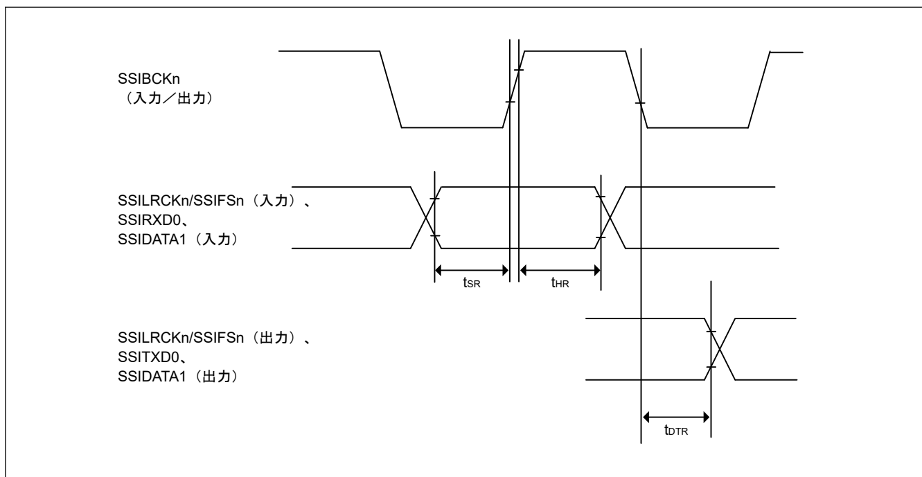
図 60.87 SSICR.BCKP = 0 の場合の SSIE データ送受信タイミング
