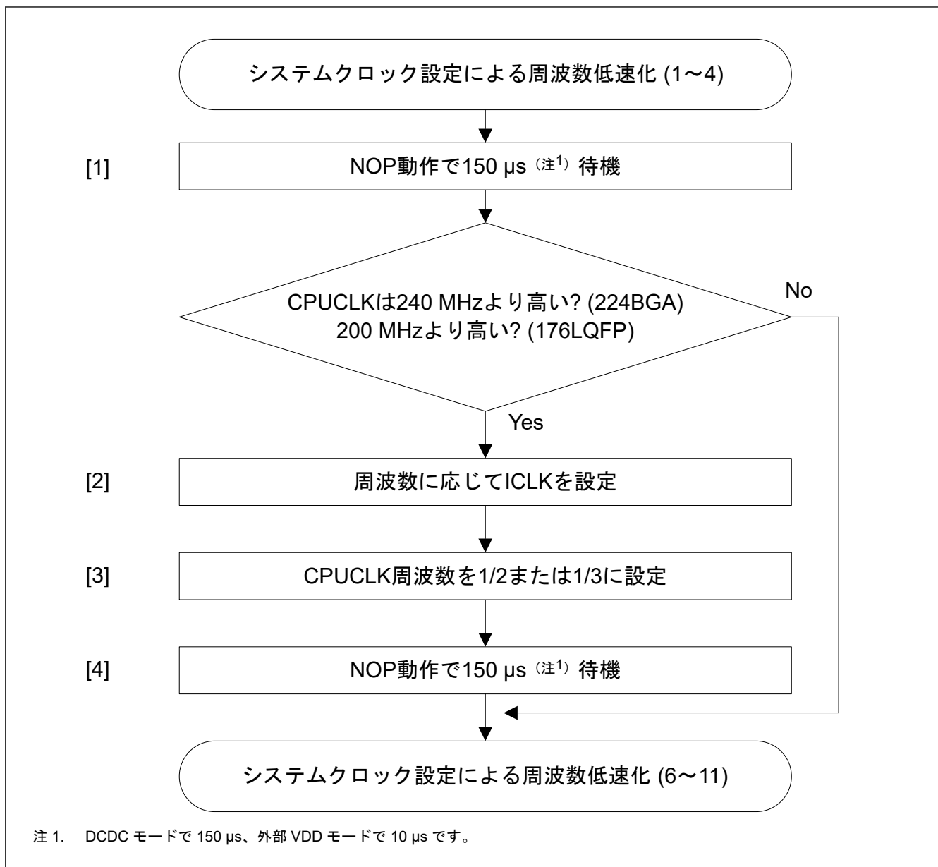
図 8.15 システムクロック設定の追加フロー（システムクロックソースおよび CPUCLK として PLL を使用し周波数を低速化する場合）
