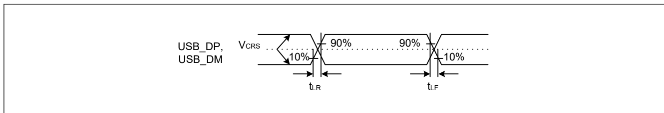
図 60.107 Low-speed モードにおける USB_DP、USB_DM の出力タイミング
