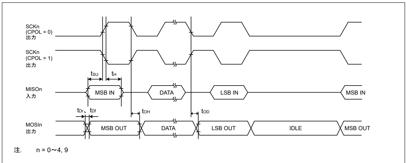
図 60.53 SCI 簡易 SPI モードタイミング (マスタ、CPHA = 0)
