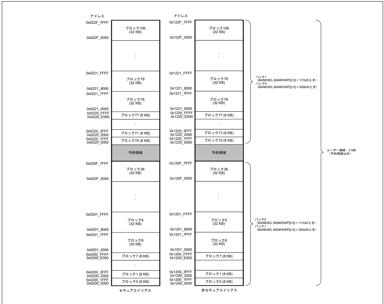
図 52.3 デュアルモードでのコードフラッシュメモリのマップ
