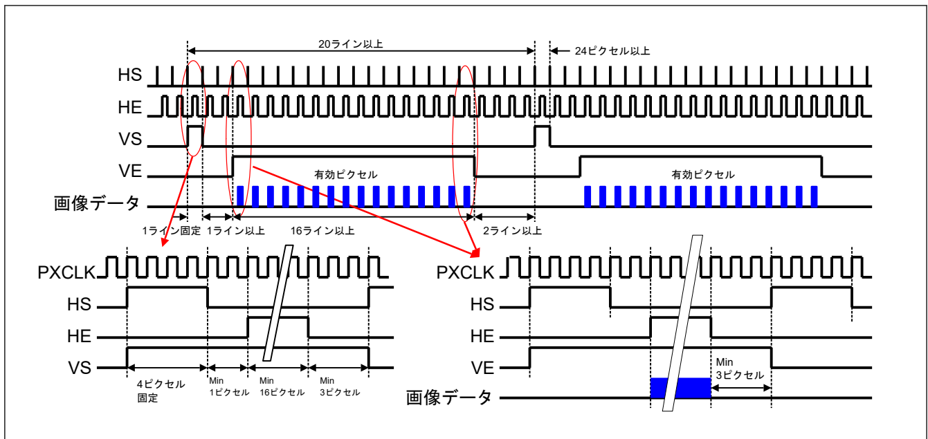
図 56.23 GLCDC 内の画像データキャリア信号
