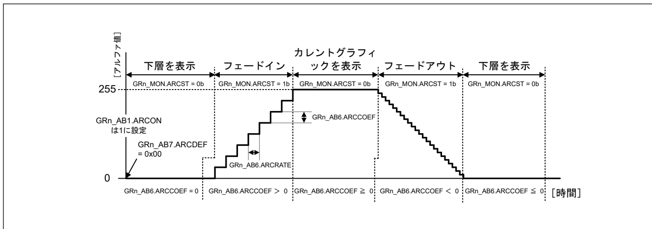
図 56.11 アルファ値の変化
