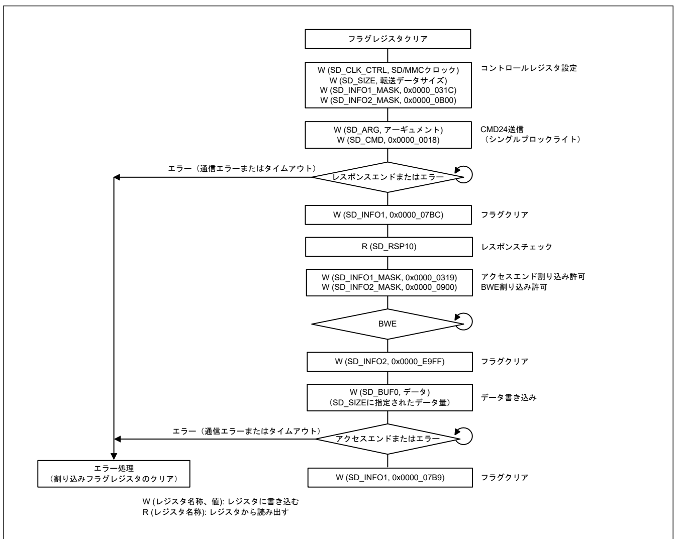
図 40.12 シングルブロックライト動作の例
