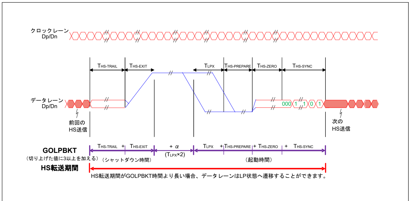
図 58.2 データレーンでの LP モードの最小期間
