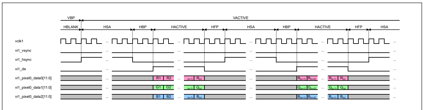
図 58.12 VBP 終了と VACTIVE 開始 (RGB)
