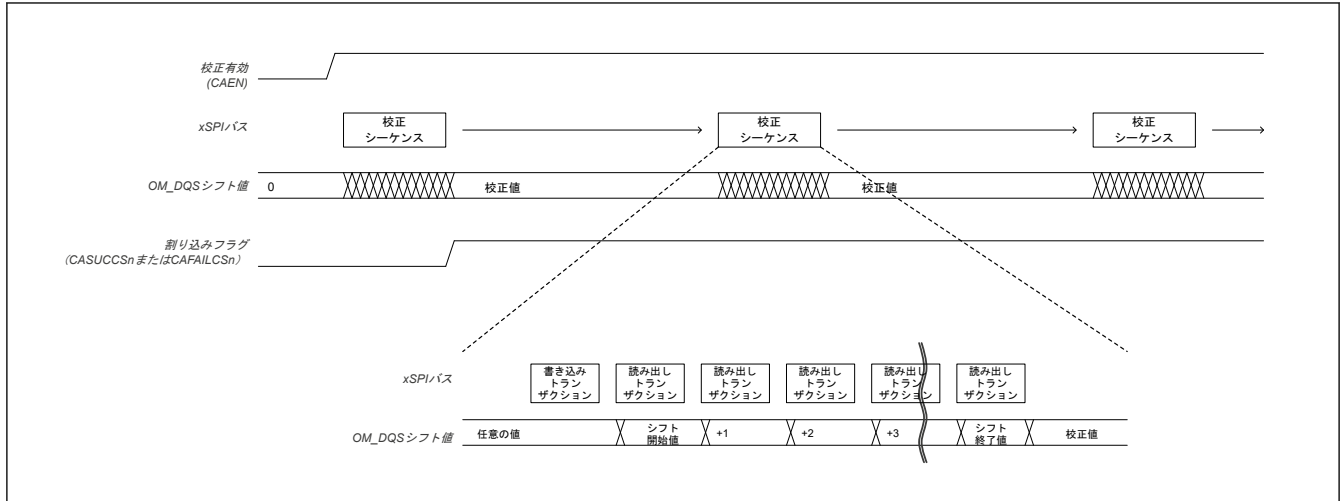
図 37.11 自動校正
