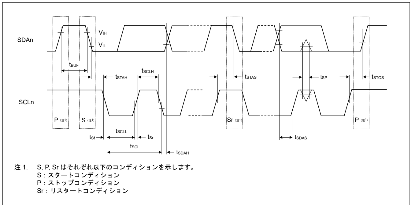
図 60.71 I 2 C バスインタフェース入出力タイミング
