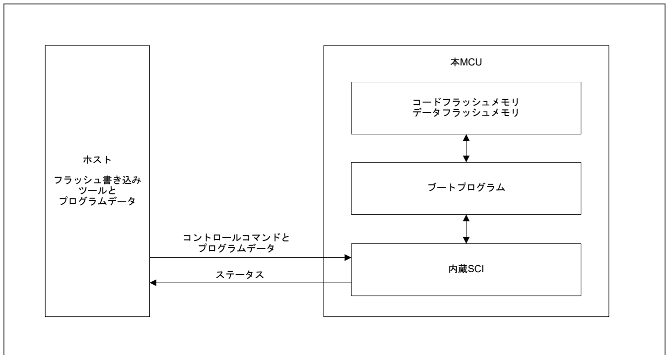
図 44.43 ブートモード（SCI インタフェース）時のシステム構成
