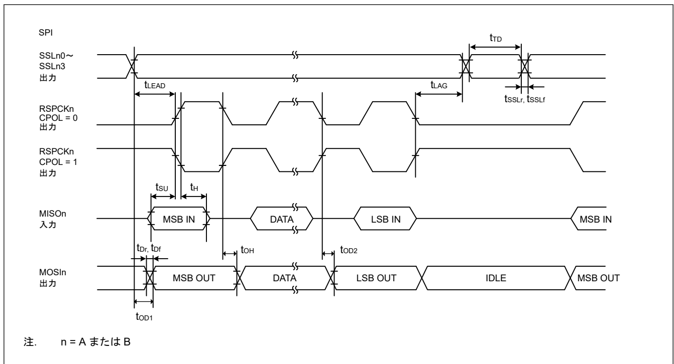
図 47.34 CPHA = 0 の場合におけるマスタの SPI タイミング
