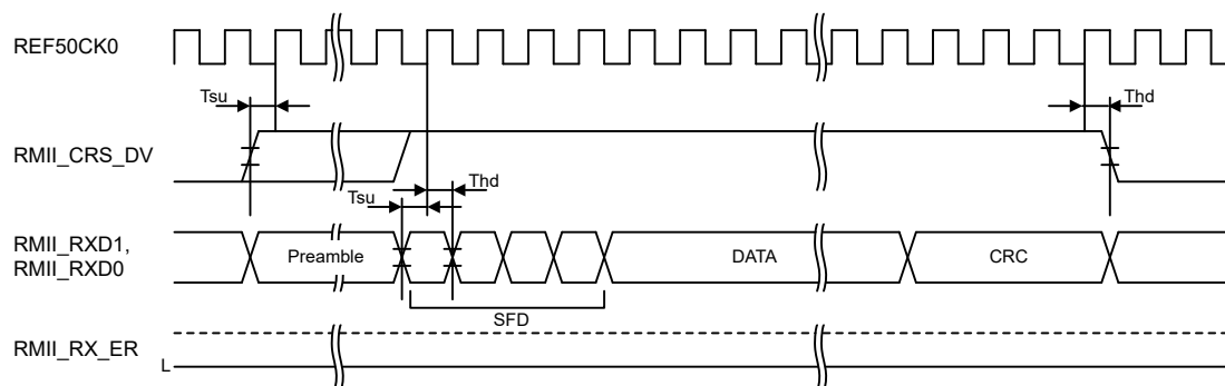
図 47.51 正常動作時の RMII 受信タイミング
