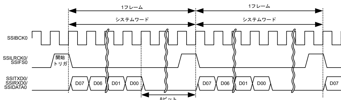
図 34.39 モノラルフォーマットにおけるショートフレーム（パディングあり、システムワード長 > データワード長）
