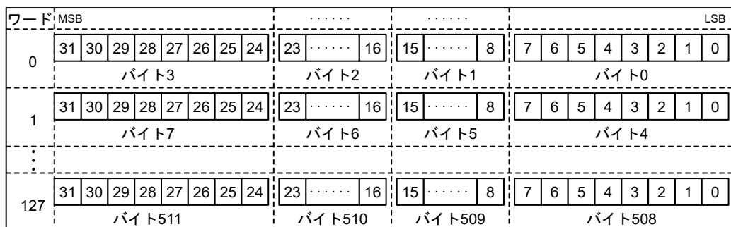
図 35.4 SD_BUF 格納データ
