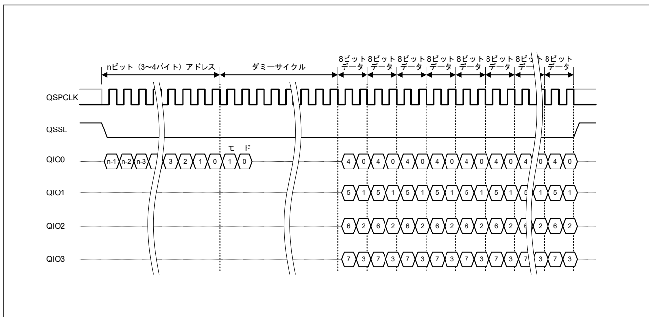
図 33.26 拡張 SPI プロトコルでの XIP モードファストリード Quad 出力バスサイクル
