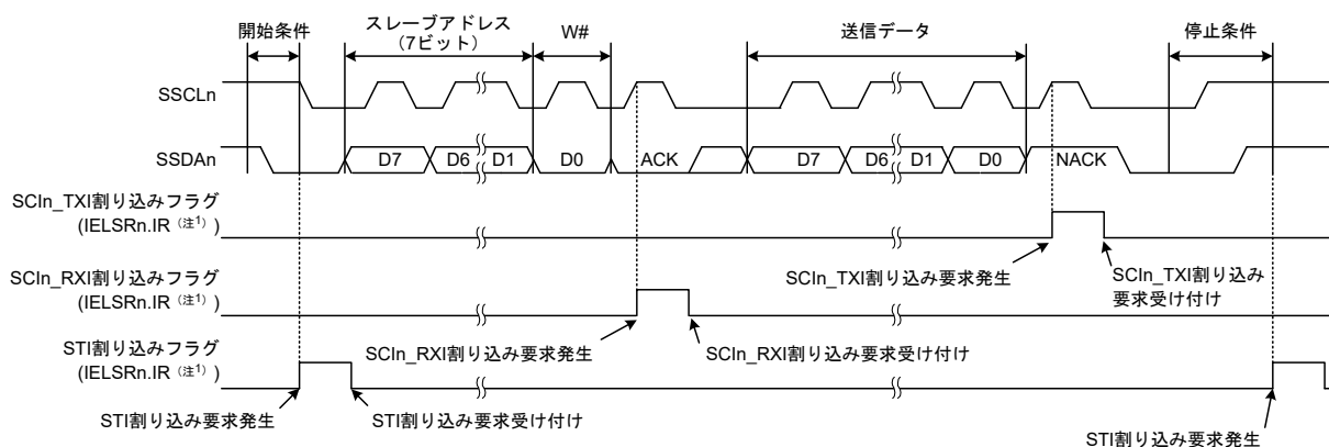
図 29.94 簡易 IIC モードにおけるマスタ送信の動作例 2 (7 ビットスレーブアドレス、ACK 割り込み、NACK 割り込み使用時)
