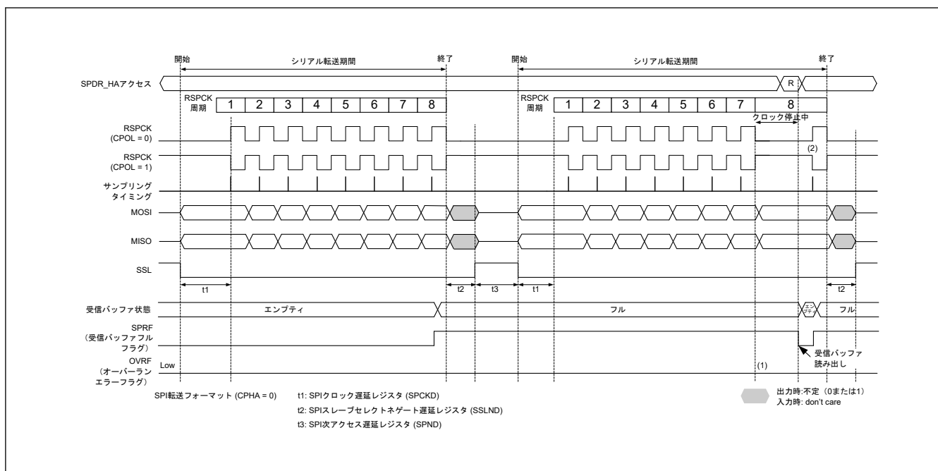
図 32.39 マスターモードの受信バッファフルの状態でのシリアル転送が継続するときのクロック停止波形 (CPHA = 0)
