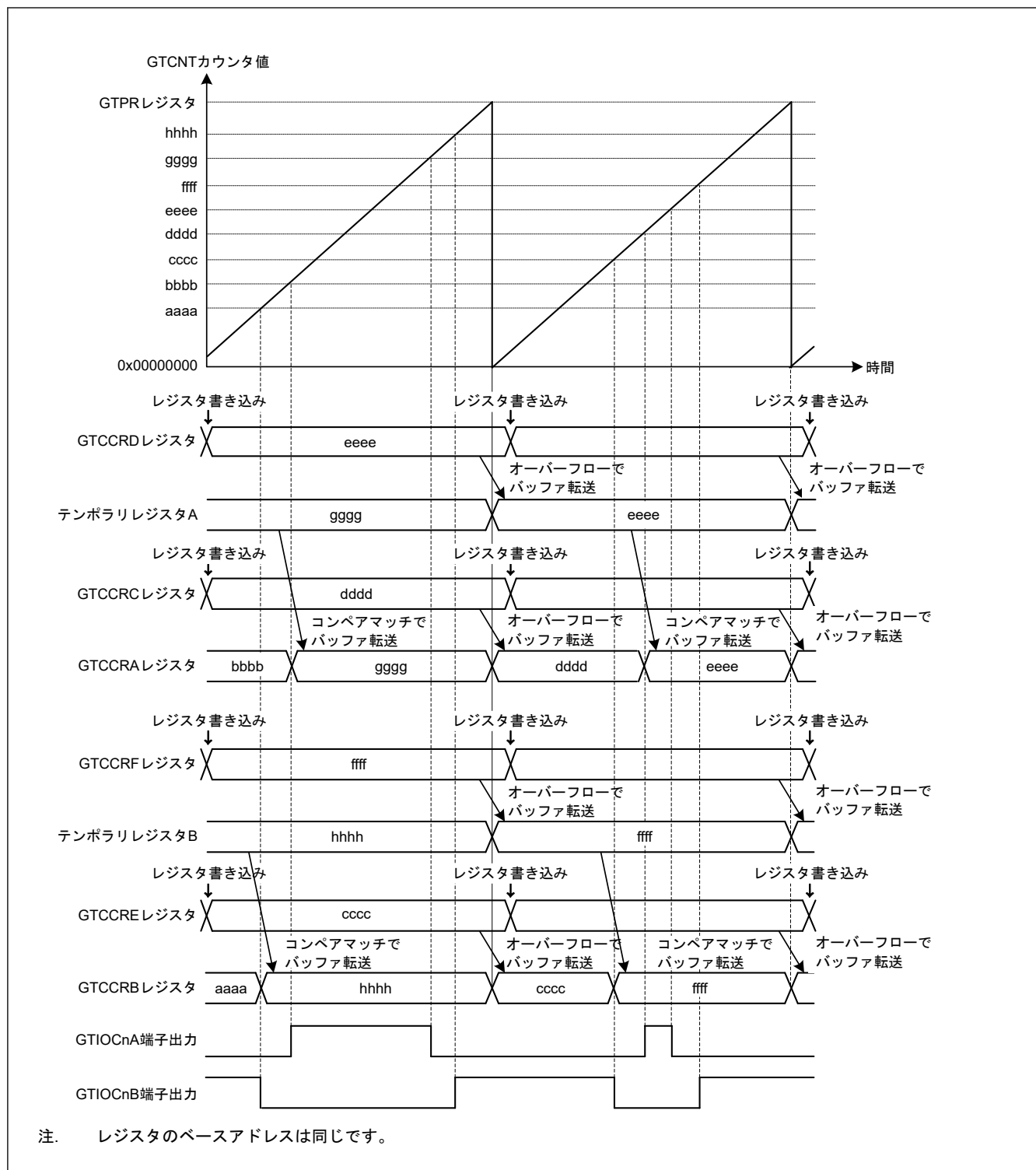
図 21.20 のこぎり波ワンショットパルスモードの動作例 (アップカウント、カウントスタート時に GTIOcNA 端子 = Low 出力/GTIOcNB 端子 = High 出力、GTCCRd/GTCCRb レジスタのコンペアマッチ時にトグル出力、周期の終わりで出力保持の場合)
