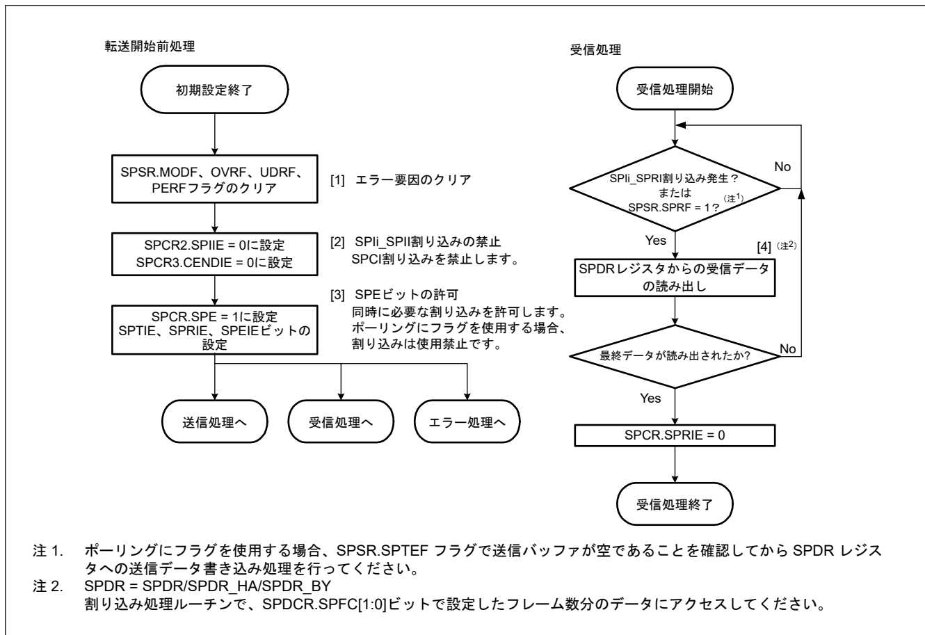
図 32.53 スレーブモードでの送信フロー
