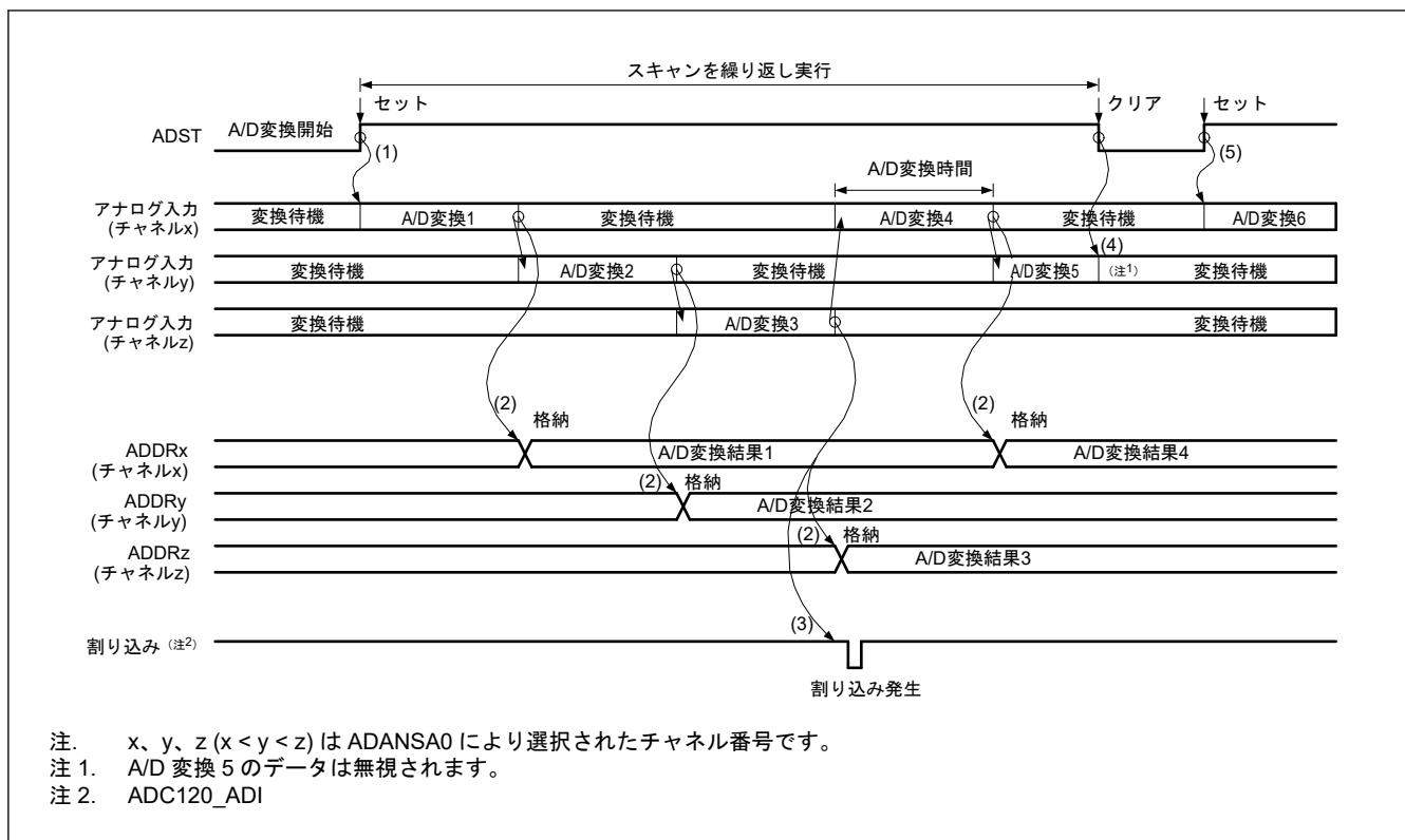
図 39.12 連続スキャンモードの基本動作例（アナログ入力（チャネル x~z）選択）
