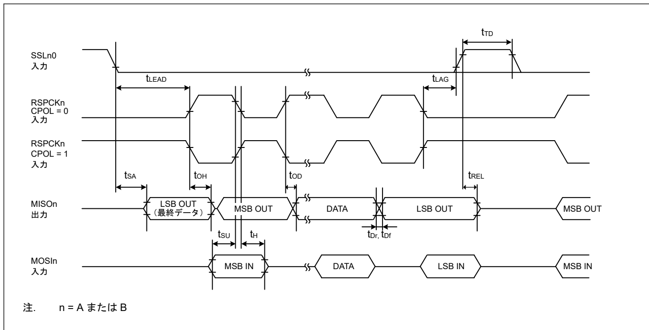
図 47.39 CPHA = 1 の場合におけるスレーブの SPI タイミング
