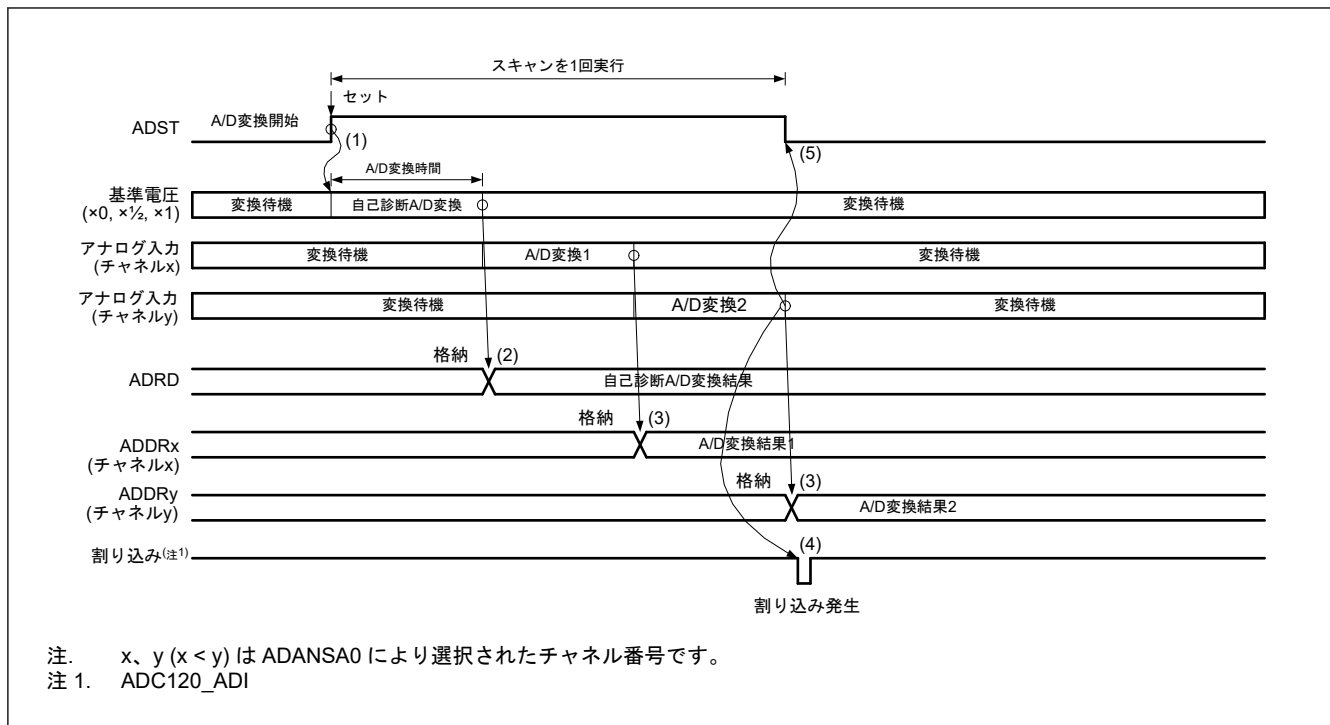
図 39.8 シングルスキャンモードの基本動作例（アナログ入力（チャネル x、y）選択+自己診断）
