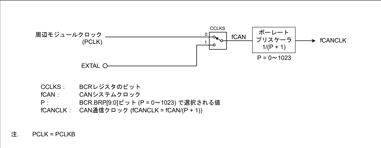
図 31.11 CAN クロック発振器のブロック図
