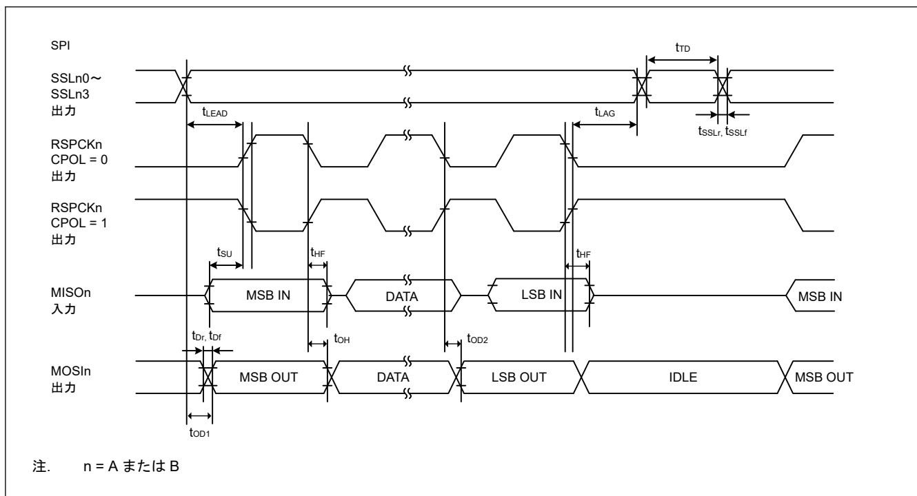
図 47.35 CPHA = 0 で、PCLKA/2 にビットレートが設定されている場合におけるマスタの SPI タイミング
