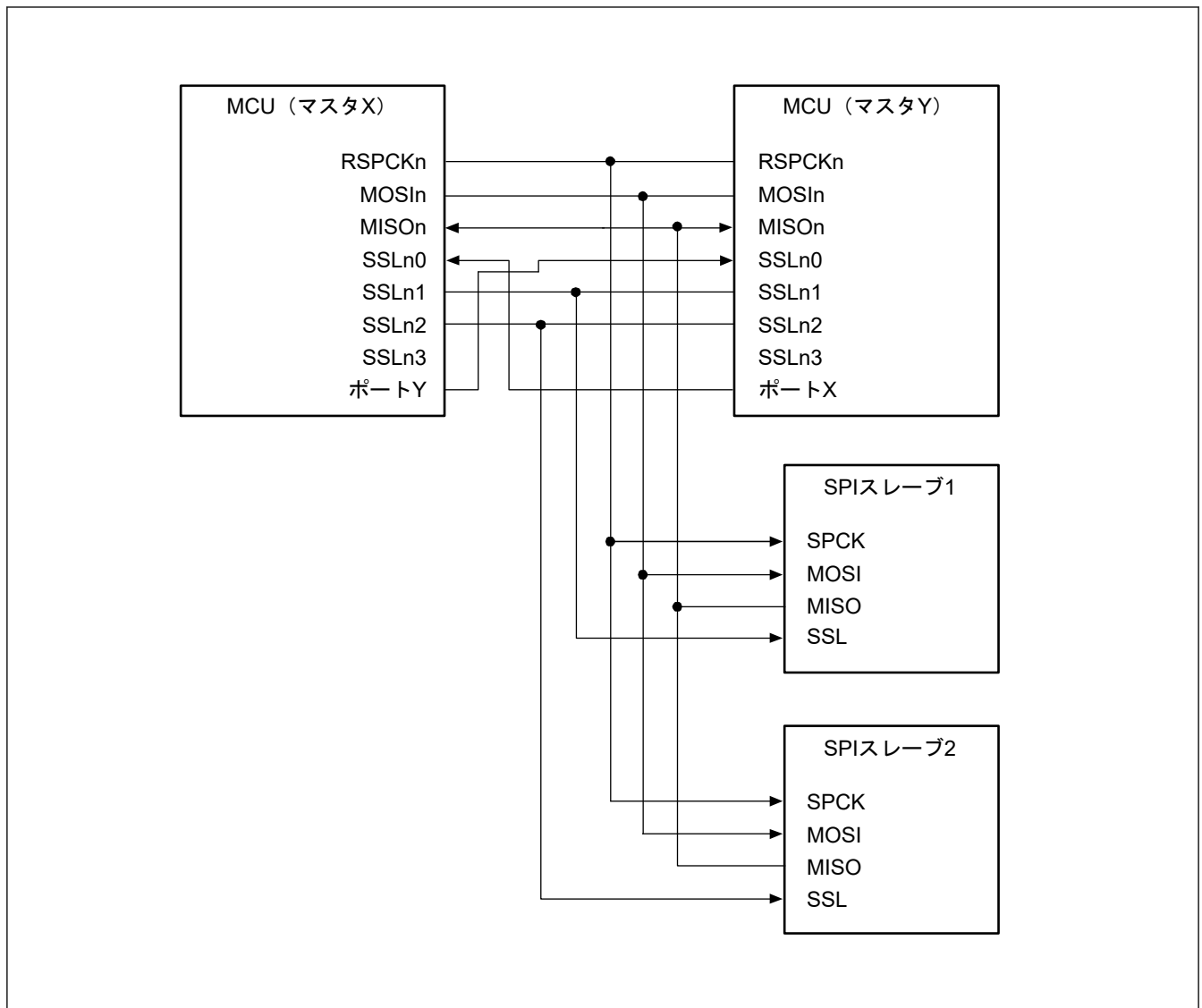
図 32.10 マルチマスタとマルチスレーブの構成例 (MCU はマスタ)
