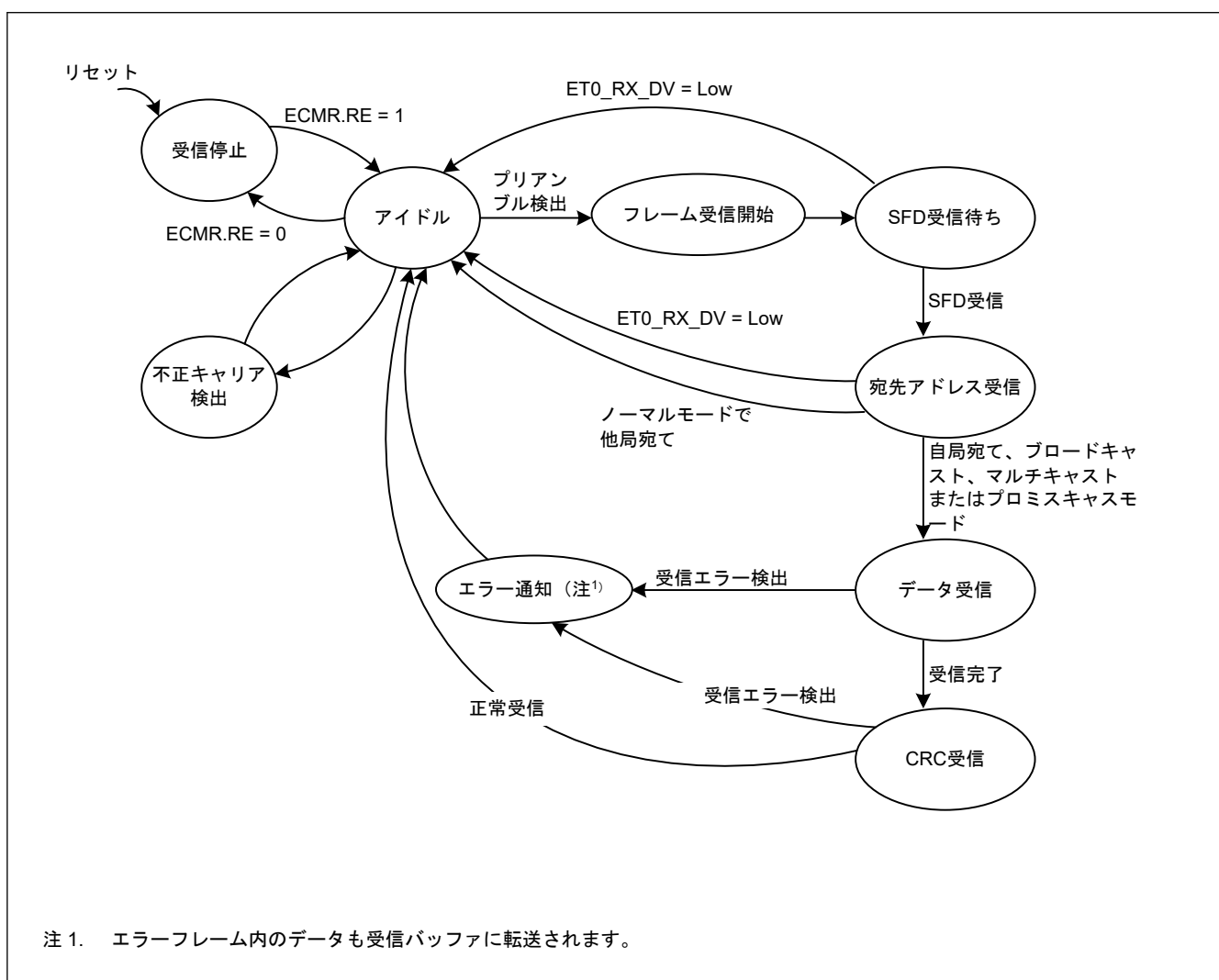
図 26.4 ETHERC 送信部の状態遷移
