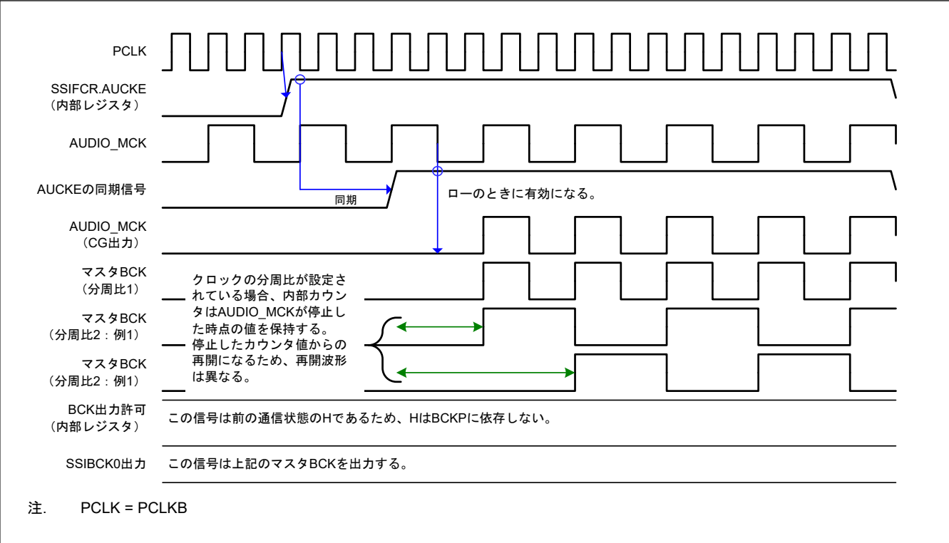
図 34.27 通信停止からマスターモード通信開始までの動作のタイミング図
