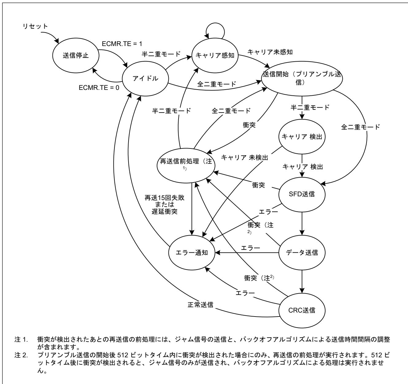
図 26.3 ETHERC 送信部の状態遷移
