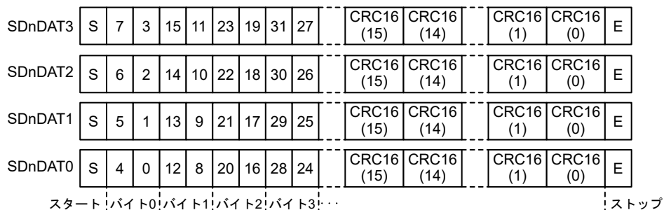
図 35.3 4 ビット幅モードの SDnDAT
