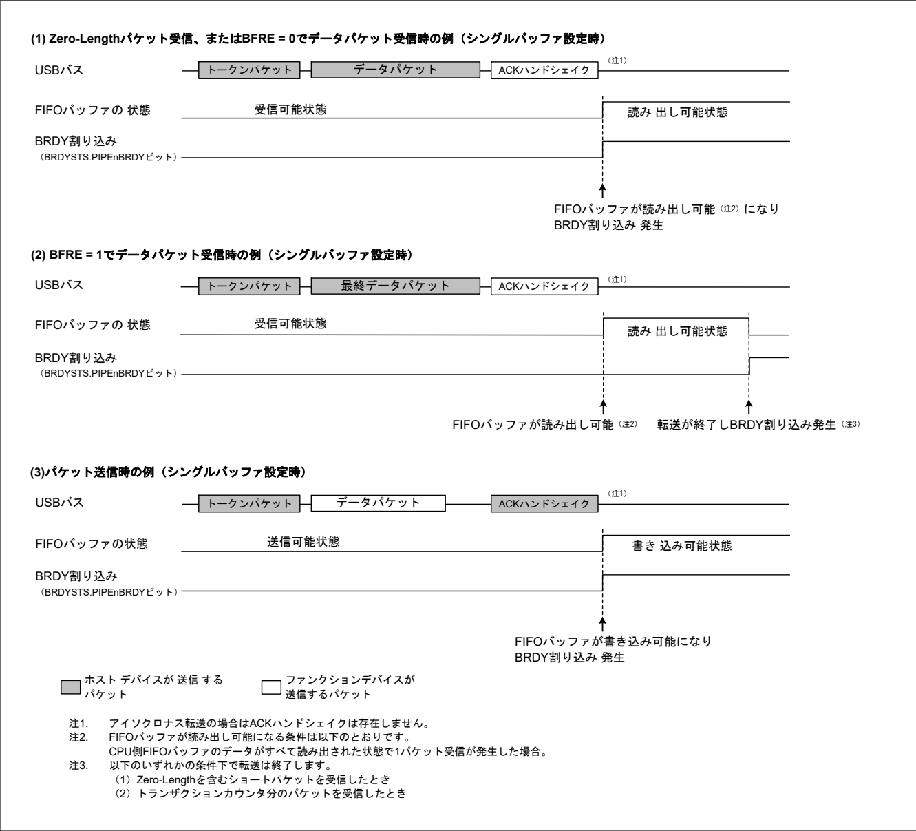
図 28.12 BRDY 割り込み発生タイミング INTSTS0.BRDY ビットがクリアされる条件は、表 28.18 に示すように、SOFCFG.BRDYM ビットの設定値によって異なります。
