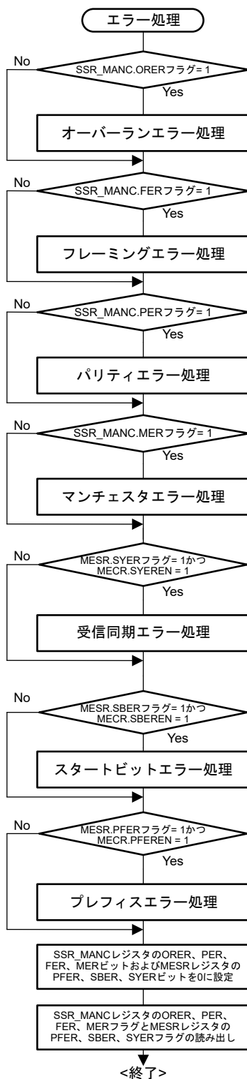
図 29.62 マンチェスタモードにおけるシリアル受信フローチャートの例（エラー処理）
