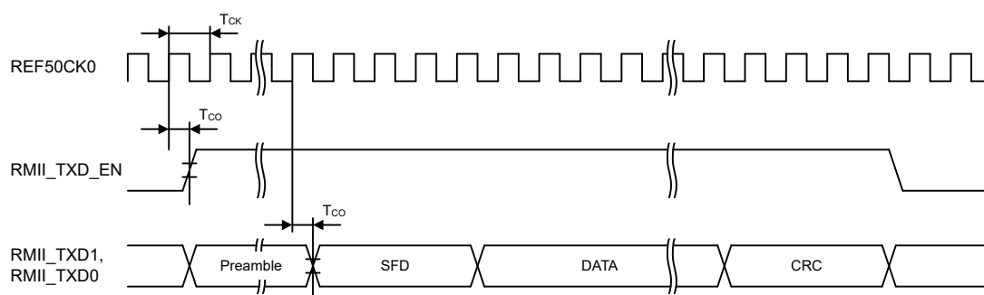
図 47.50 RMII 送信タイミング
