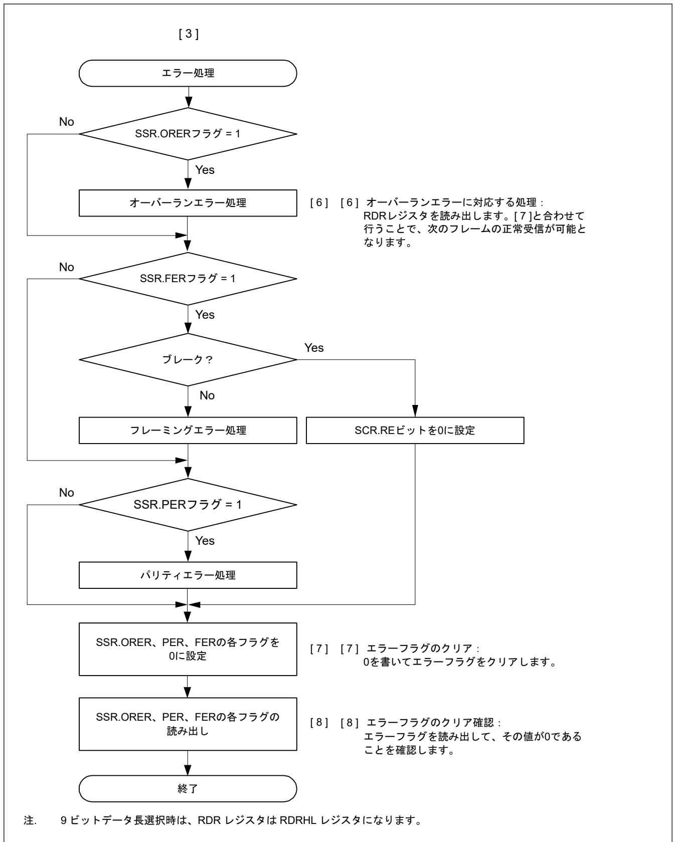
図 29.21 調歩同期式モードにおけるシリアル受信のフローチャート例（非 FIFO 選択、アドレス一致検出無効時） (2)
