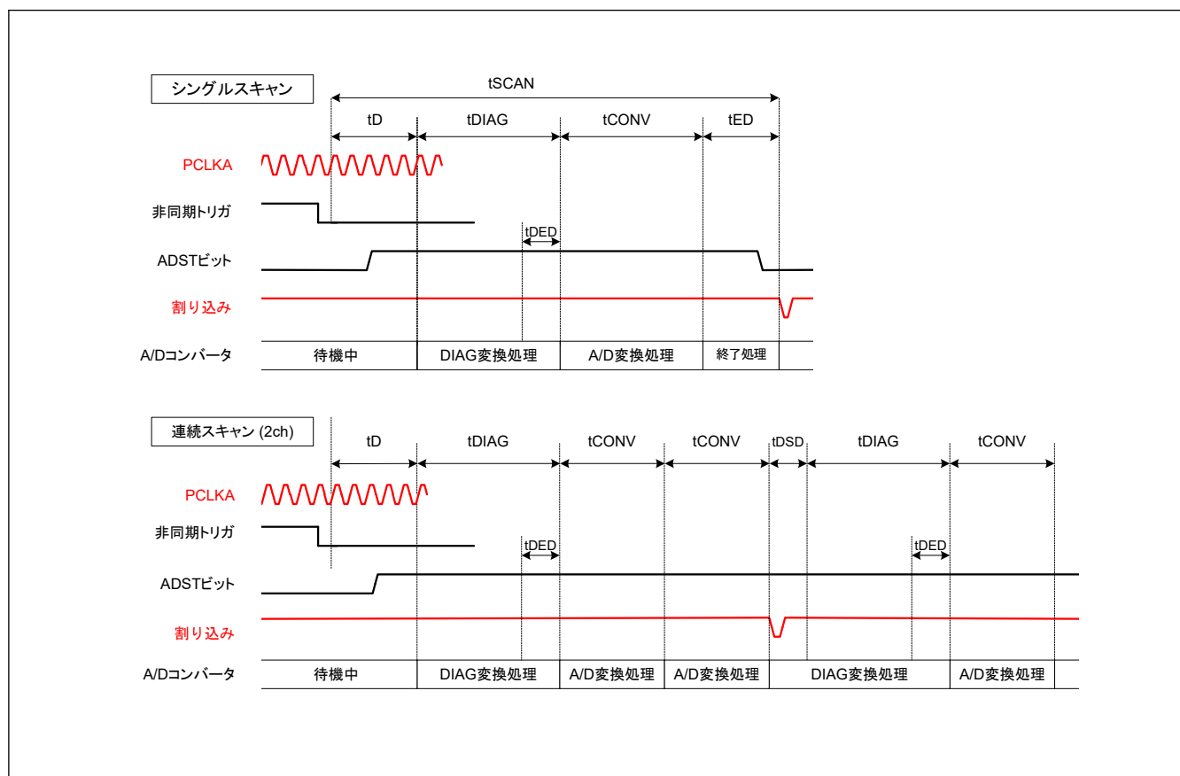
図 39.27 スキャン変換のタイミング (非同期トリガ入力 (ADTRG0) 起動の場合)
