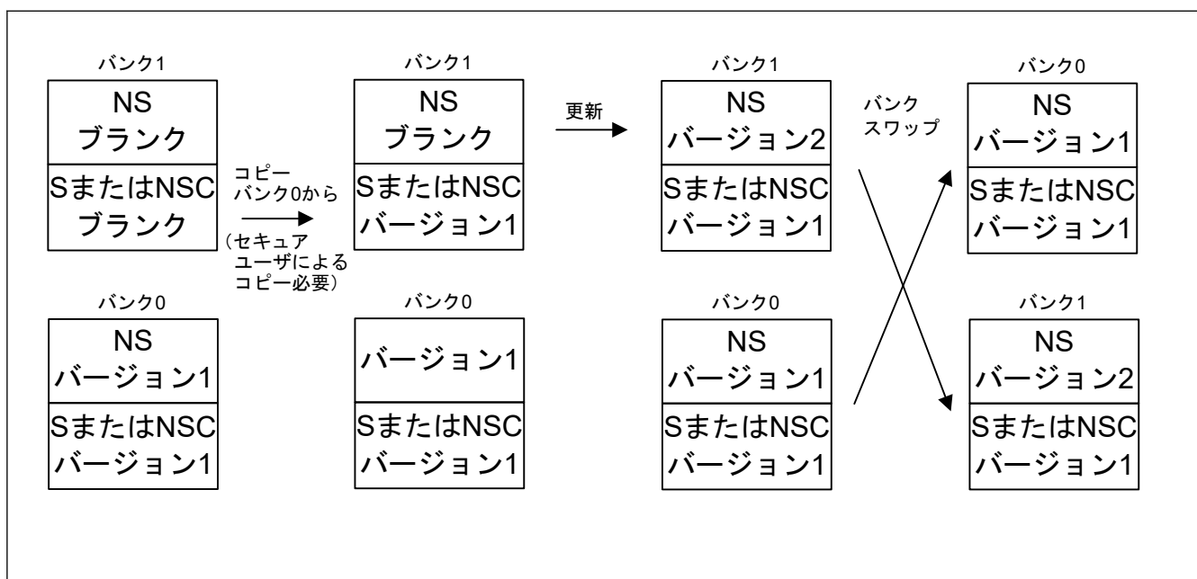
図 46.5 非セキュア領域のフィールドアップデートフロー
