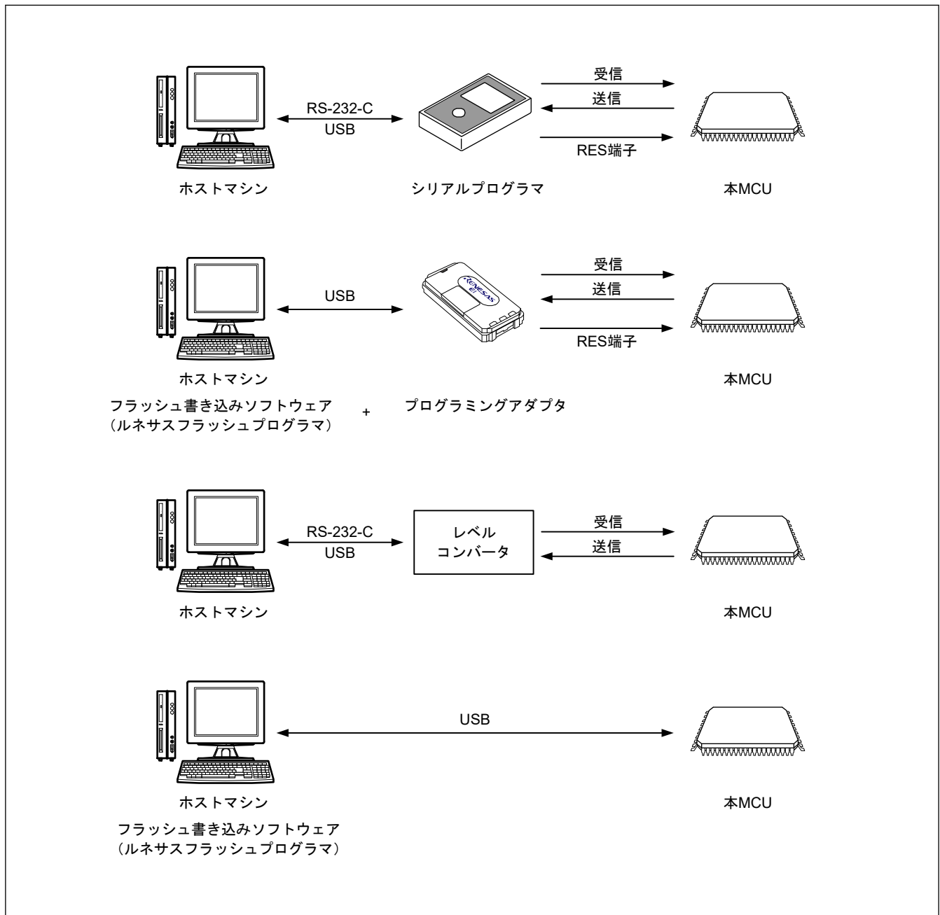
図 44.45 フラッシュメモリを書き換えるための環境
