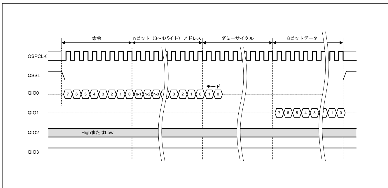
図 33.4 シングル SPI プロトコル例 (ファストリード)
