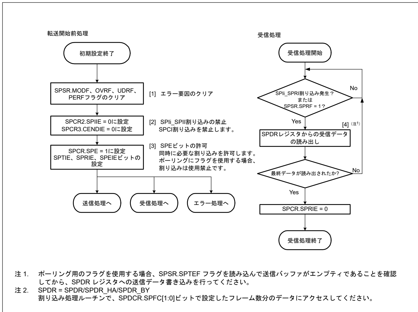
図 32.54 スレーブモードでの受信フロー
