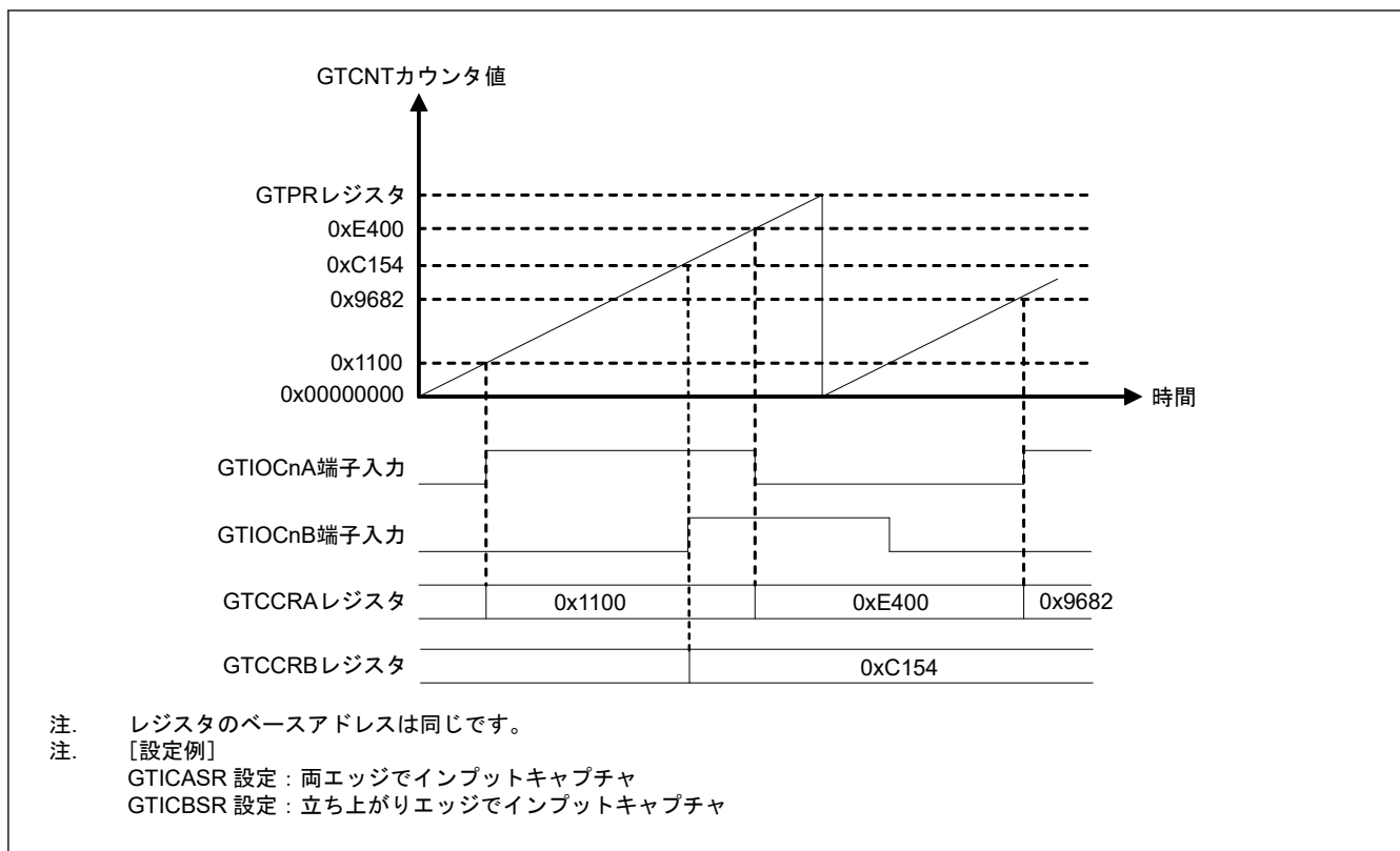
図 21.10 インพุットキャプチャ動作例
