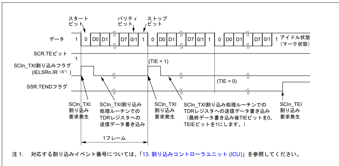
図 29.13 調歩同期式モードにおけるシリアル送信の動作例 (3) (8 ビットデータ／パリティあり／1 ストップビット／CTS 機能不使用／送信中～送信終了時)
