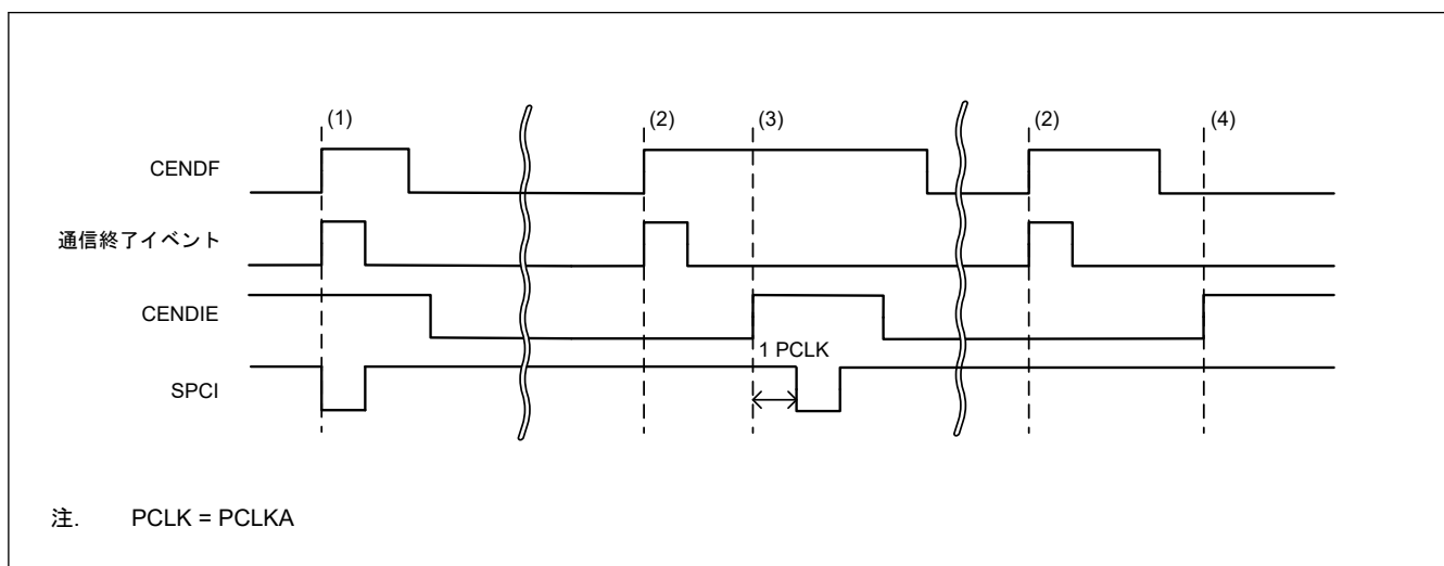
図 32.36 通信終了割り込みの動作例（イネーブル制御）
