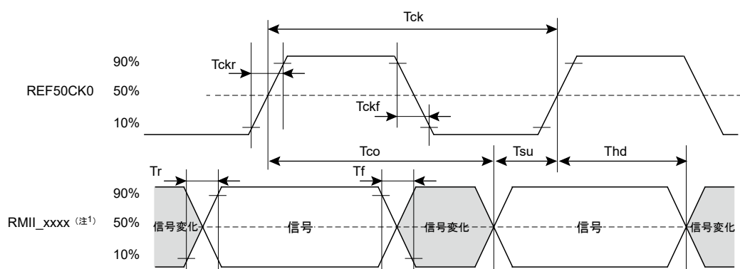
図 47.49 REF50CK0、RMII の信号タイミング
