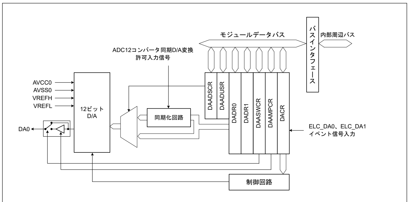
図 40.1 DAC12 のブロック図
