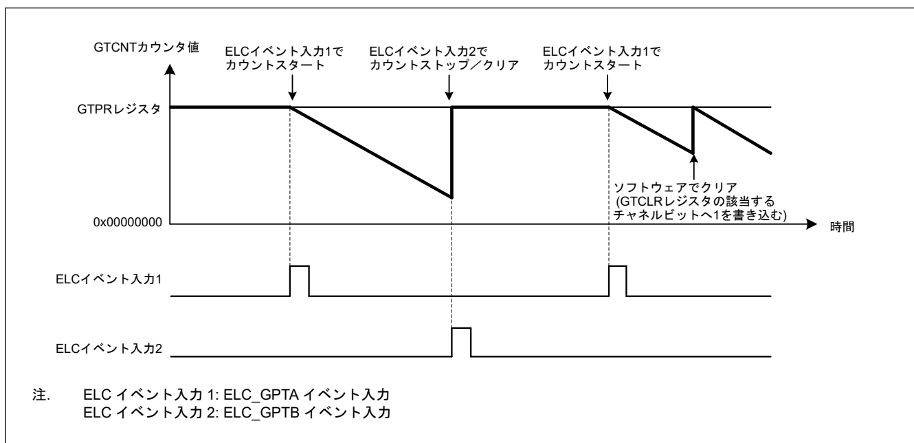
図 20.99 ハードウェア要因によるカウントクリア動作例 (のこぎり波ダウンカウント、ELC_GPTA 入力でスタート、ELC_GPTB 入力でストップ/クリアの場合)
