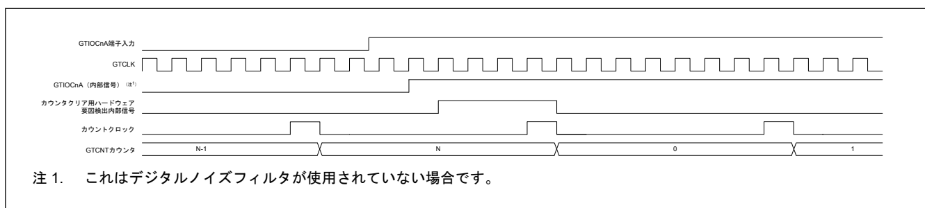
図 20.102 GTIOChA 端子入力の立ち上がりエッジに対応するカウンタクリアの動作タイミング例 (GTCLK 信号の分周により生成されるクロック信号の周期計数中)
