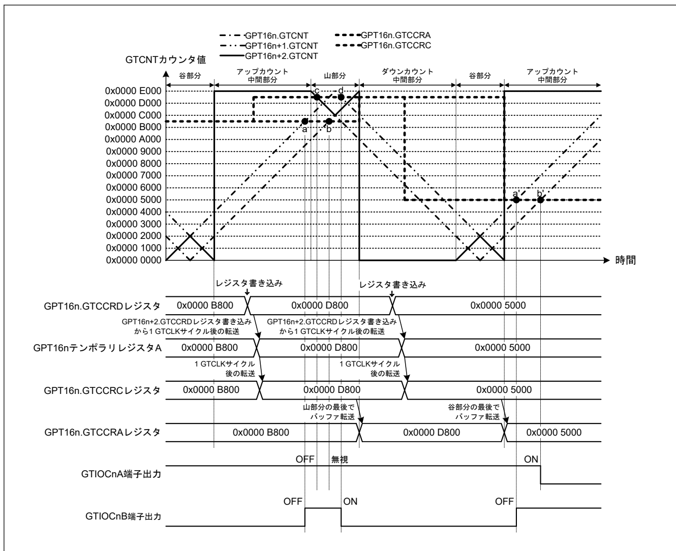
図 20.57 相補 PWM モードでのコンペアマッチ発生シーケンス動作例 (相補 PWM モード 3 シングルバッファ動作、アップカウントの GTCCRA レジスタコンペアマッチ時: GTIOCnA 端子 = Low/GTIOCnB 端子 = High、ダウンカウントの GTCCRA レジスタコンペアマッチ時: GTIOCnA 端子 = High/GTIOCnB 端子 = Low、デッドタイム値: 0x0000 2000、コンペアマッチ発生順序: a → c → b → d) (n = 0)
