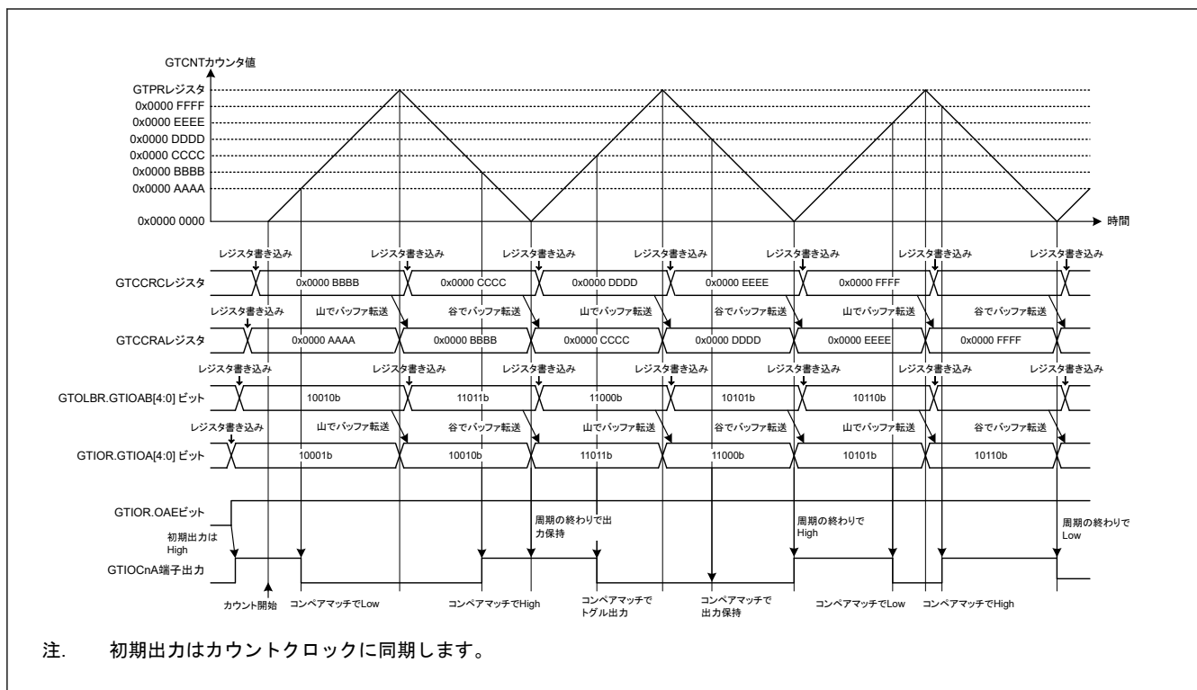
図 20.36 GTIOA ビットおよび GTIOB ビットのバッファ操作例 (三角波 PWM モード 2、山および谷でバッファ転送)
