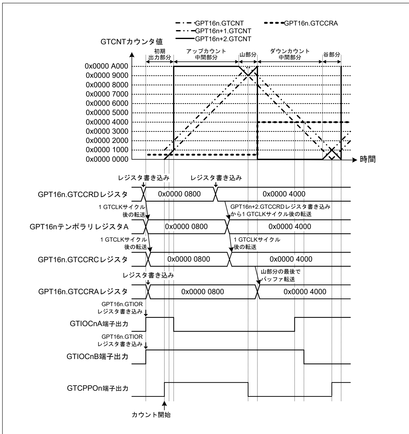
図 20.68 相補 PWM モード初期出力動作例 (相補 PWM モード 1 動作、アップカウントの GTCCRA レジスタコンペアマッチ時: GTIOCN A 端子 = Low/GTIOCN B 端子 = High、ダウンカウントの GTCCRA レジスタコンペアマッチ時: GTIOCN A 端子 = High/GTIOCN B 端子 = Low、デッドタイム値: 0x0000 1000、初期 GTCCRA レジスタ値がデッドタイム値以下の場合) (n = 0)
