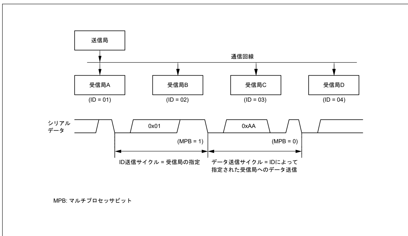
図 24.26 マルチプロセッサフォーマットを使用した通信例（データ 0xAA を受信局 A に送信する場合）
