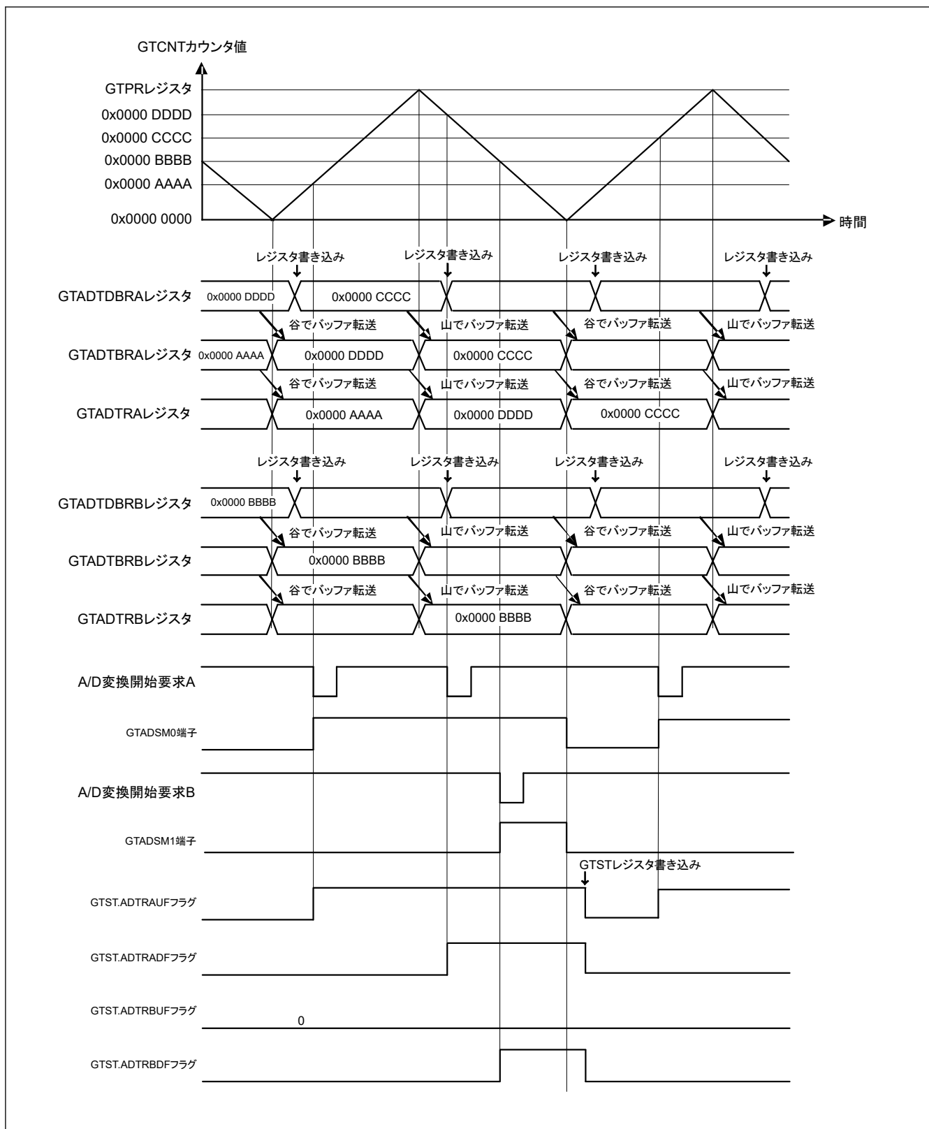
図 20.160 A/D 変換開始要求タイミング動作例 (三角波、ダブルバッファ動作、谷/山両方でバッファ転送の場合、GTADTRA レジスタはアップカウント/ダウンカウント両方で A/D 変換開始要求、GTADTRB はダウンカウントで A/D 変換開始要求、GTADSM0 端子で GTADTRA レジスタのアップカウントを監視、GTADSM1 端子で GTADTRB レジスタのダウンカウントを監視の場合)
