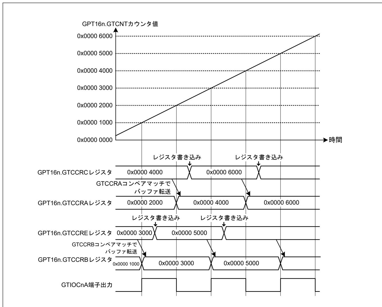
図 20.39 のこぎり波 PWM モード 2 の動作例 (GTCCRA レジスタコンペアマッチ時に Low 出力、GTCCRB レジスタコンペアマッチ時に High 出力、シングルバッファ動作、クリア設定なし) (n = 0~2)
