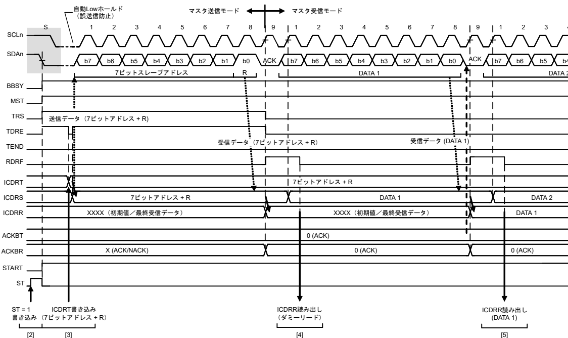
図 25.12 マスタ受信の動作タイミング (1) (7 ビットアドレスフォーマットで RDRFS = 0 の場合)
