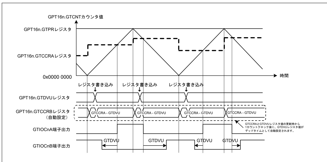
図 20.86 デッドタイム付きコンペアマッチ値の自動設定機能の動作例（三角波 PWM モード 2 または 3、GPT163 でアクティブ High の場合）
