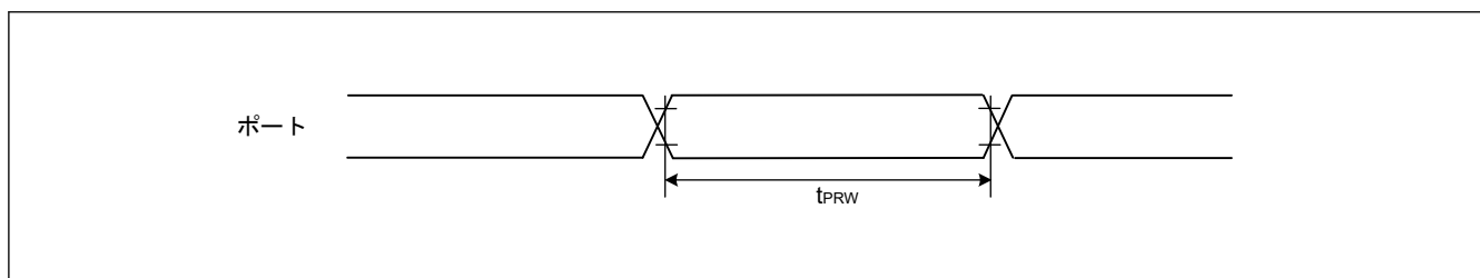
図 35.13 I/O ポート入力タイミング
