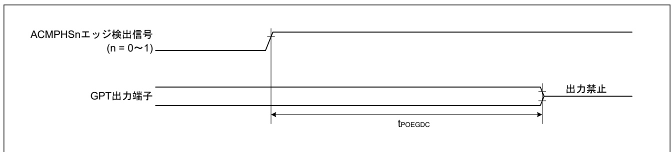
図 35.17 ACMPHS からのエッジ検出信号に対応した POEG の出力禁止時間
