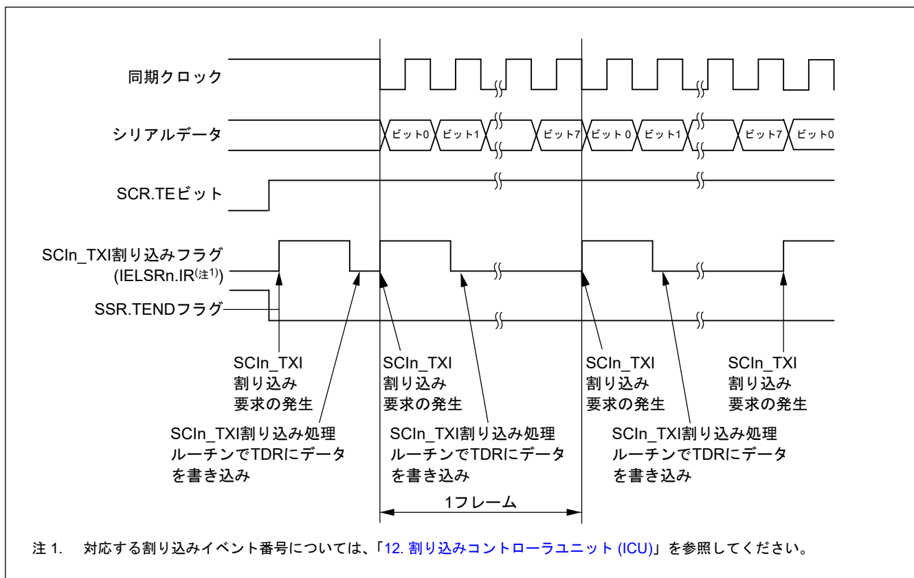
図 24.36 クロック同期式モードにおけるシリアル送信の動作例 (送信開始時に CTS 機能を使用しない場合)
