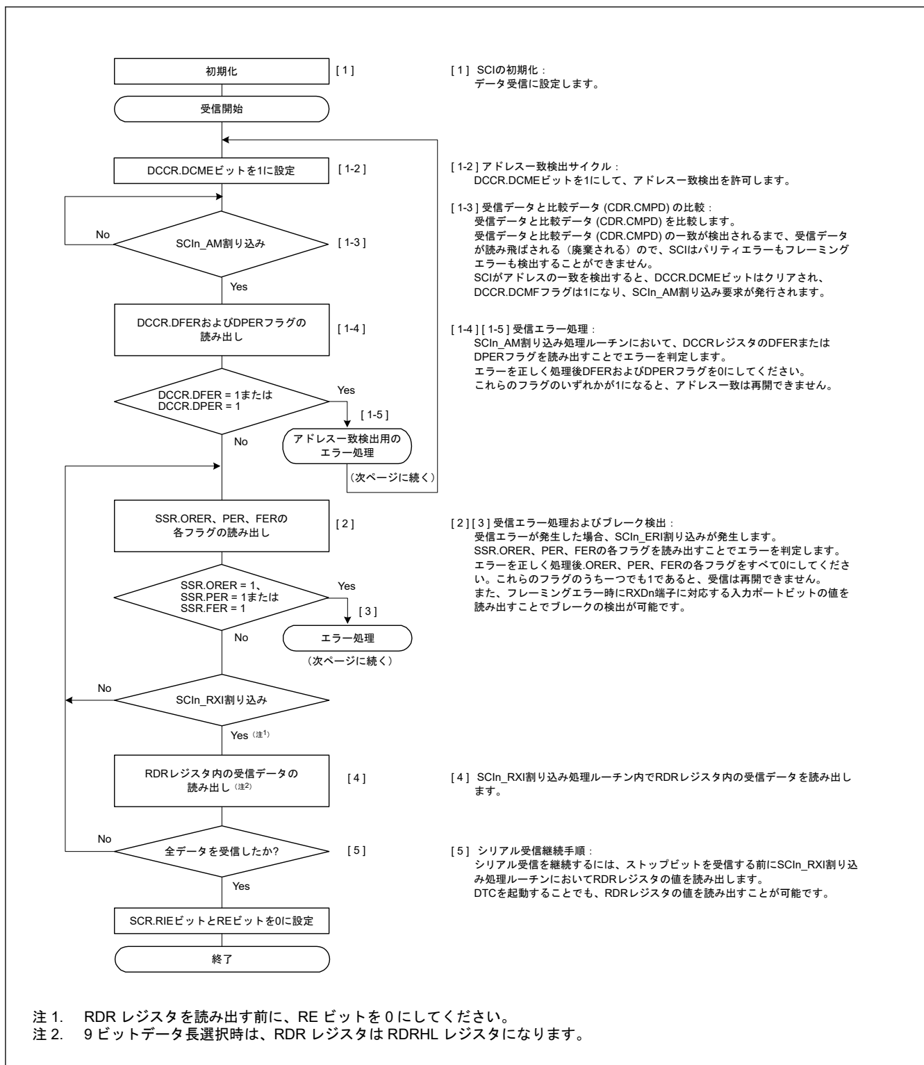
図 24.17 調歩同期式モードにおけるシリアル受信のフローチャート例（非 FIFO 選択、アドレス一致検出有効時） (1)
