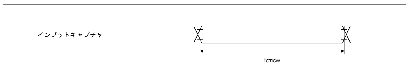
図 35.22 GPT インプットキャプチャタイミング
