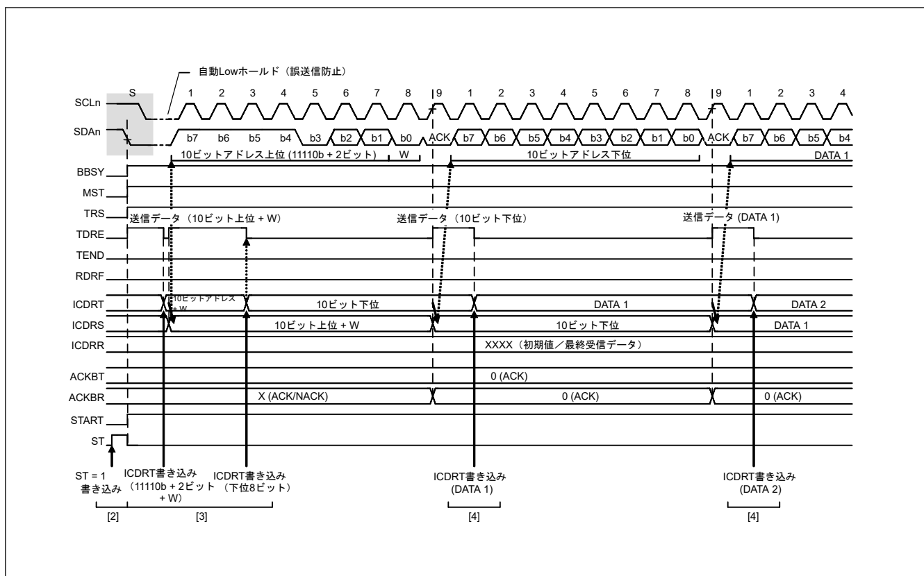
図 25.8 マスタ送信の動作タイミング (2) (10 ビットアドレスフォーマット)
