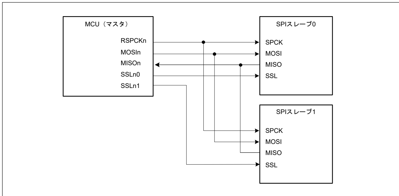
図 26.8 シングルマスタとマルチスレーブの構成例 (MCU はマスタ)
