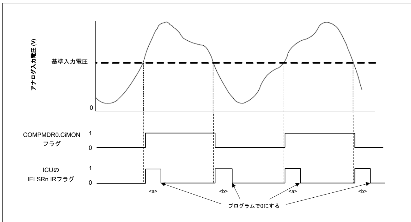
図 28.2 ACMPHS の動作例
