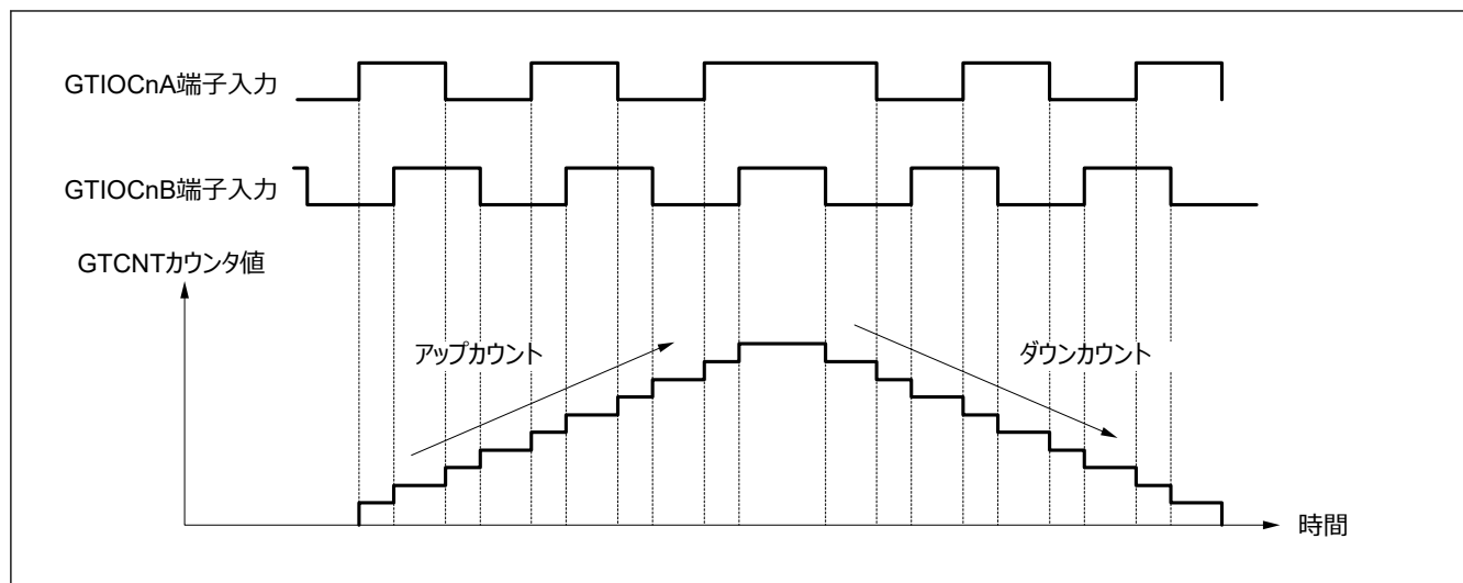
図 20.123 位相計数モード 1 の動作例
