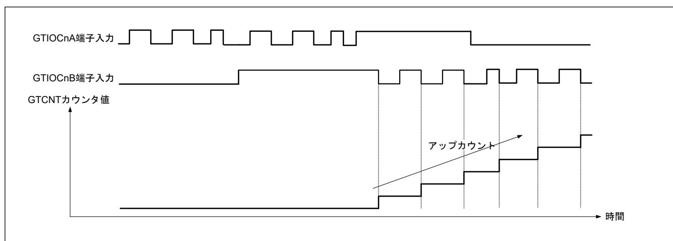
図 20.132 位相計数モード 5 の動作例 (B)
