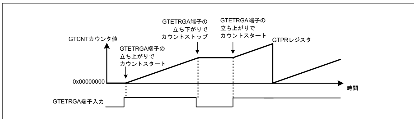
図 20.94 ハードウェア要因によるカウントスタート／ストップ動作例（GTETRGA 端子入力の立ち上がりエッジでスタート、GTETRGA 端子入力の立ち下がりエッジでストップの場合）
