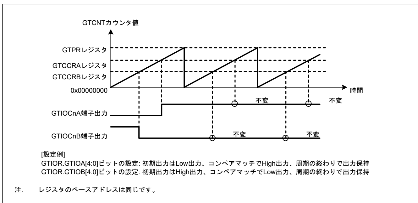
図 20.10 Low 出力/High 出力動作例
