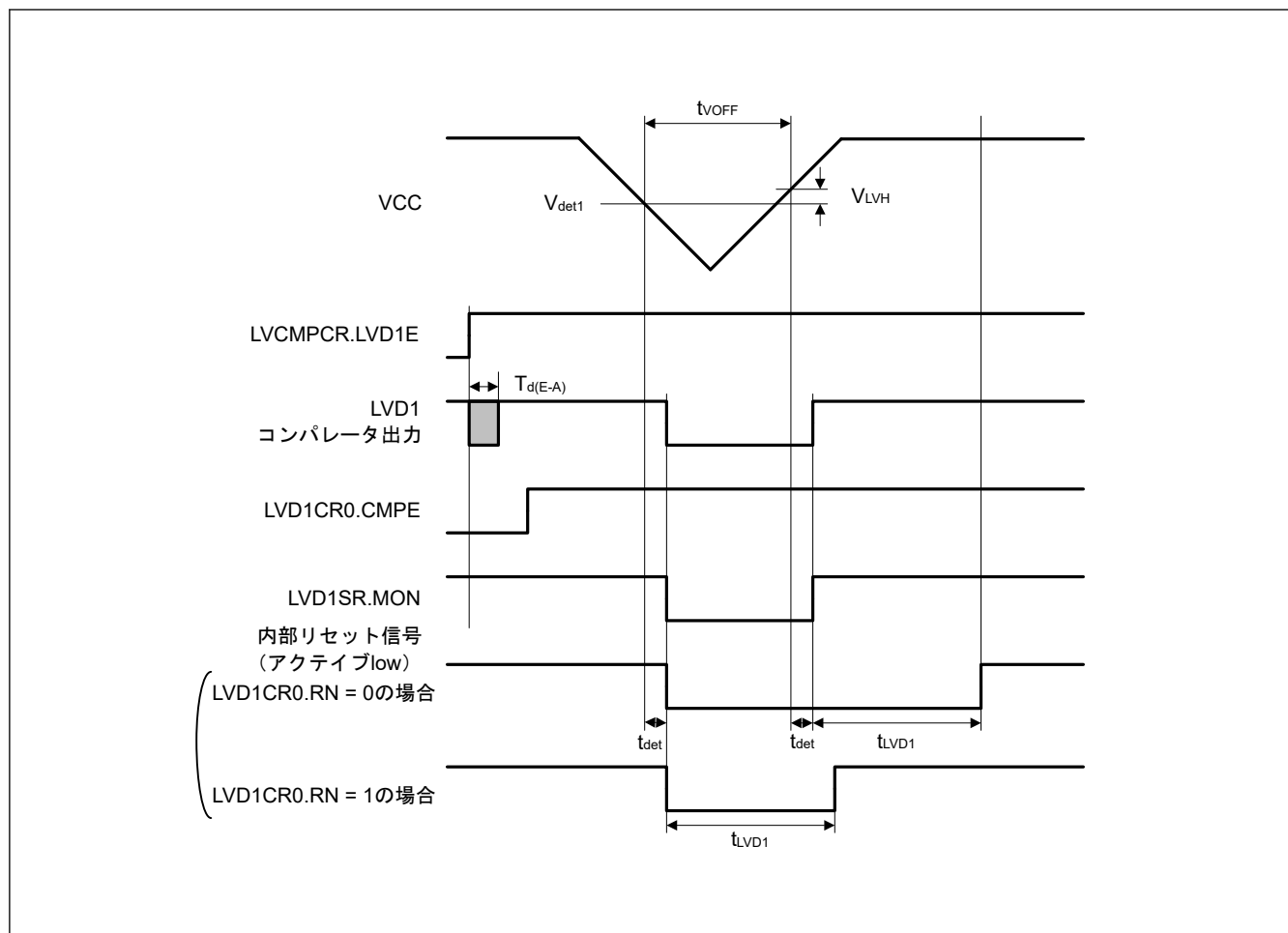
図 35.55 電圧検出回路タイミング ( V_{det1} )
