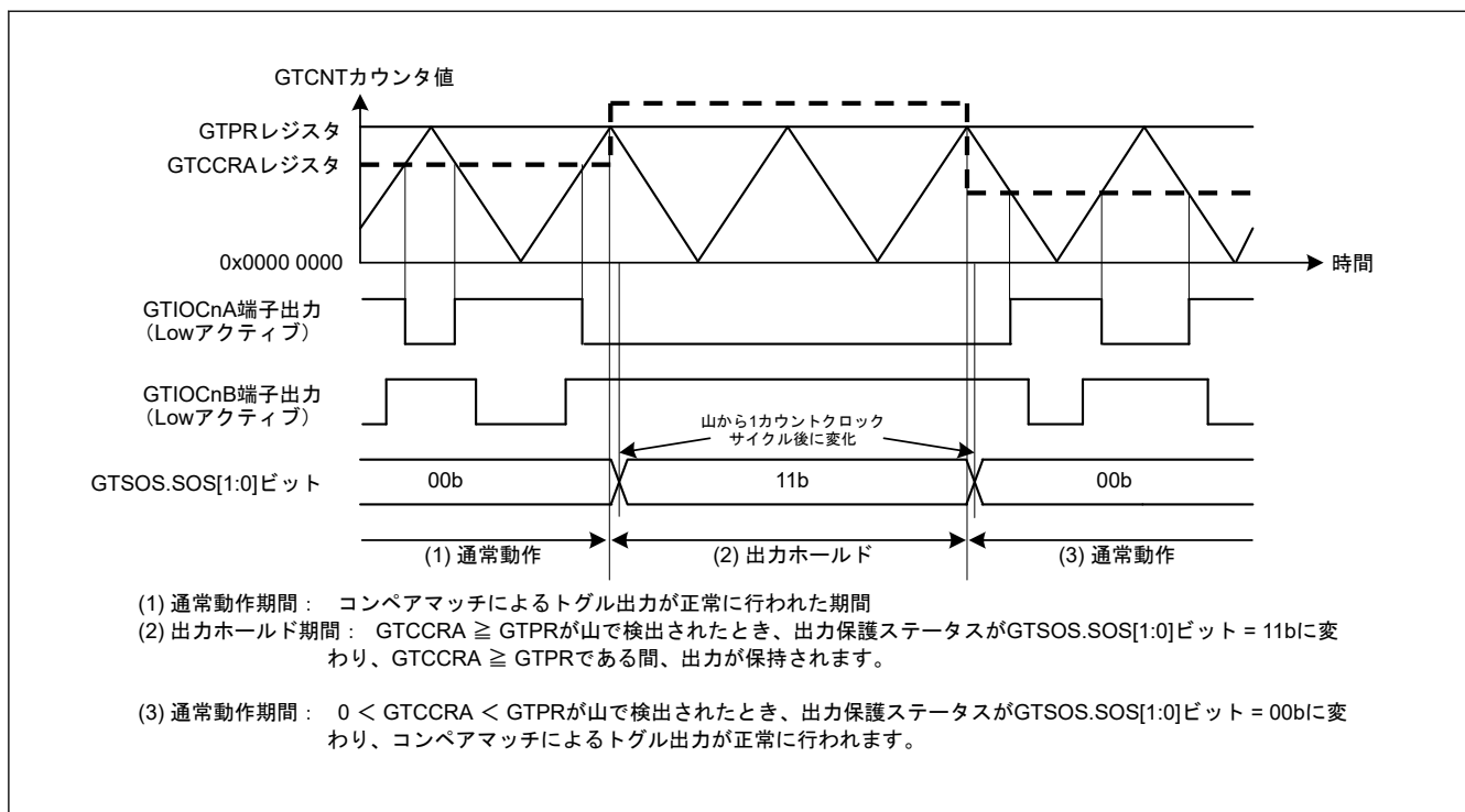
図 20.178 山でのバッファ転送中に GTCCR \geq GTPR となったときの出力保護機能の動作例 (山でのバッファ転送中に 0 < GTCCR < GTPR に復帰、アクティブレベル : Low) ( n = 0 \sim 2 )
