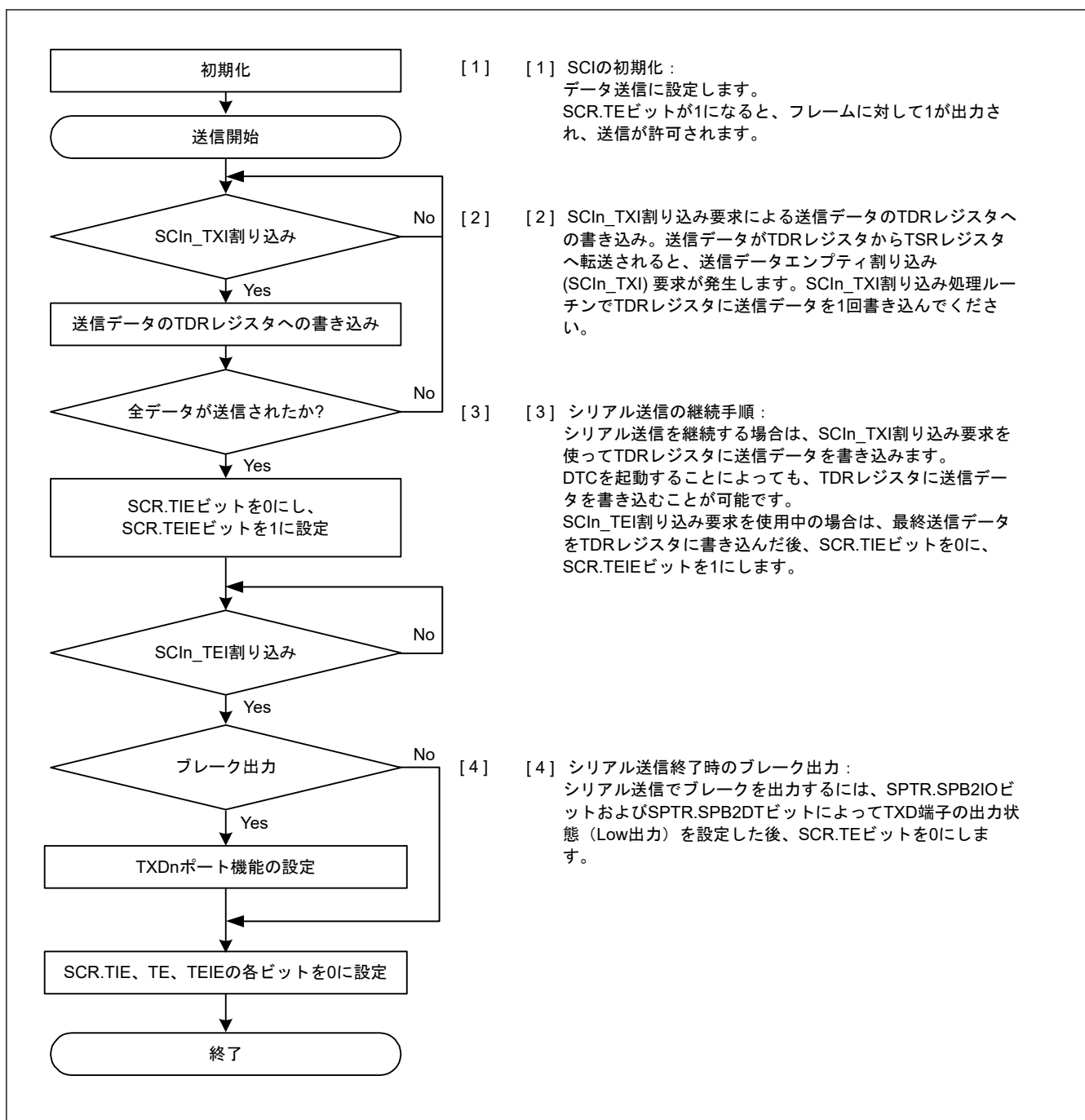
図 24.10 調歩同期式モードにおけるシリアル送信のフローチャート例 (非 FIFO 選択時)
