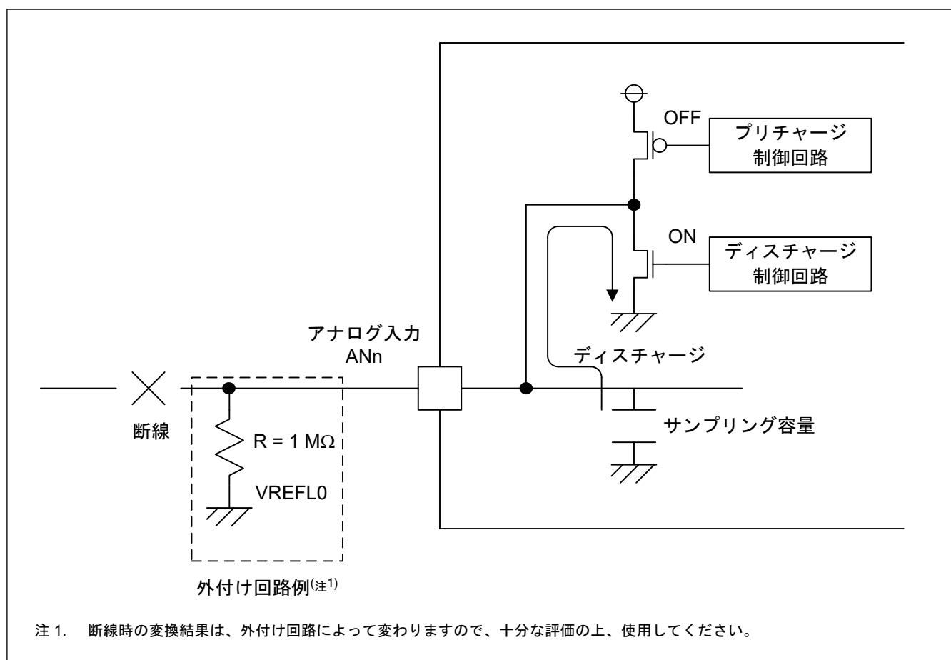
図 29.33 ディスチャージを選択した場合の断線検出例
