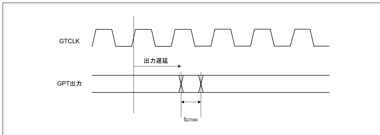
図 35.23 GPT 出力遅延スキュー
