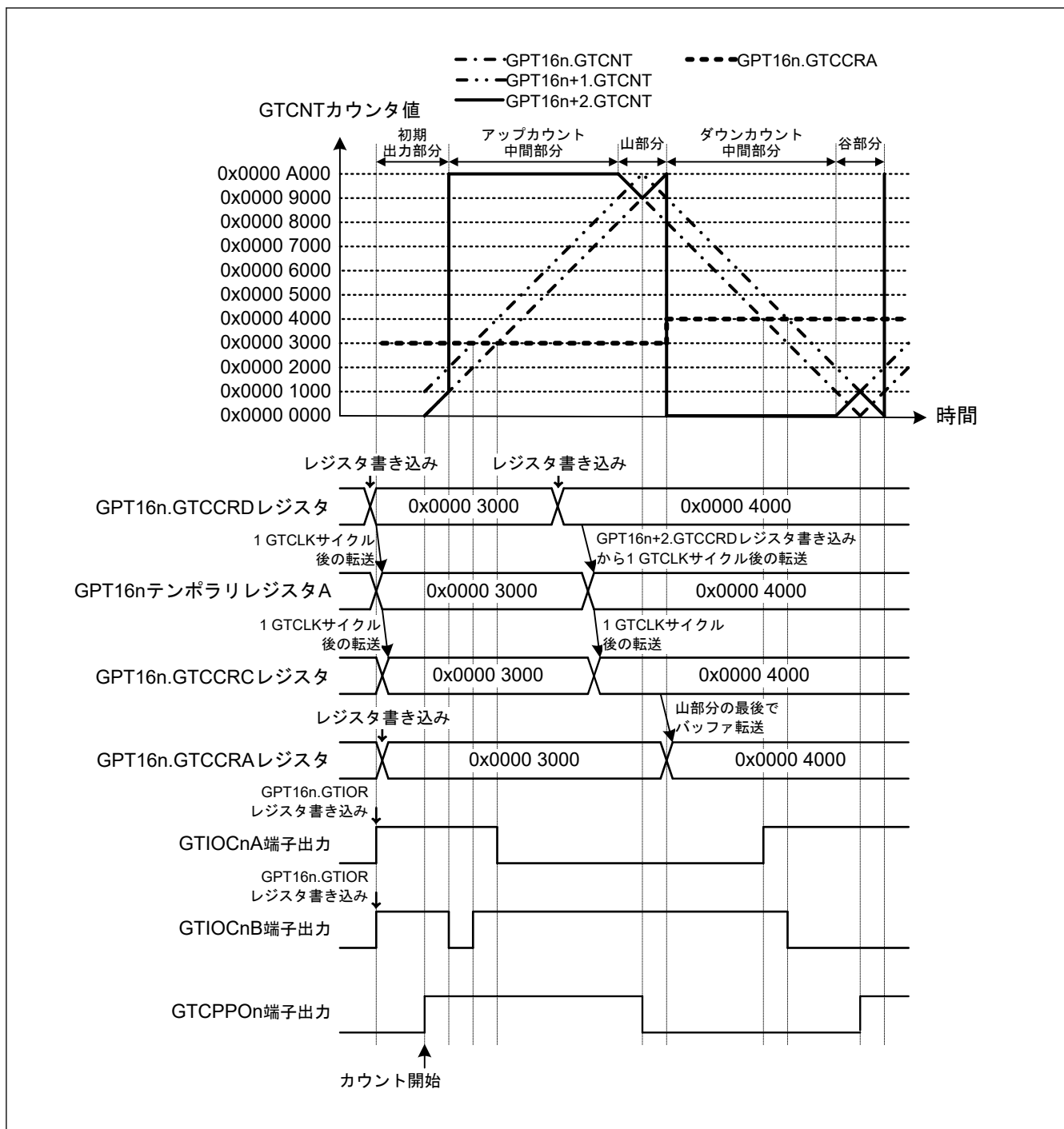
図 20.67 相補 PWM モード初期出力動作例 (相補 PWM モード 1 動作、アップカウントの GTCCRA レジスタコンペアマッチ時: GTIOCnA 端子 = Low/GTIOCnB 端子 = High、ダウンカウントの GTCCRA レジスタコンペアマッチ時: GTIOCnA 端子 = High/GTIOCnB 端子 = Low、デッドタイム値: 0x0000 1000、初期 GTCCRA レジスタ値がデッドタイム値より大きい場合) (n = 0)
