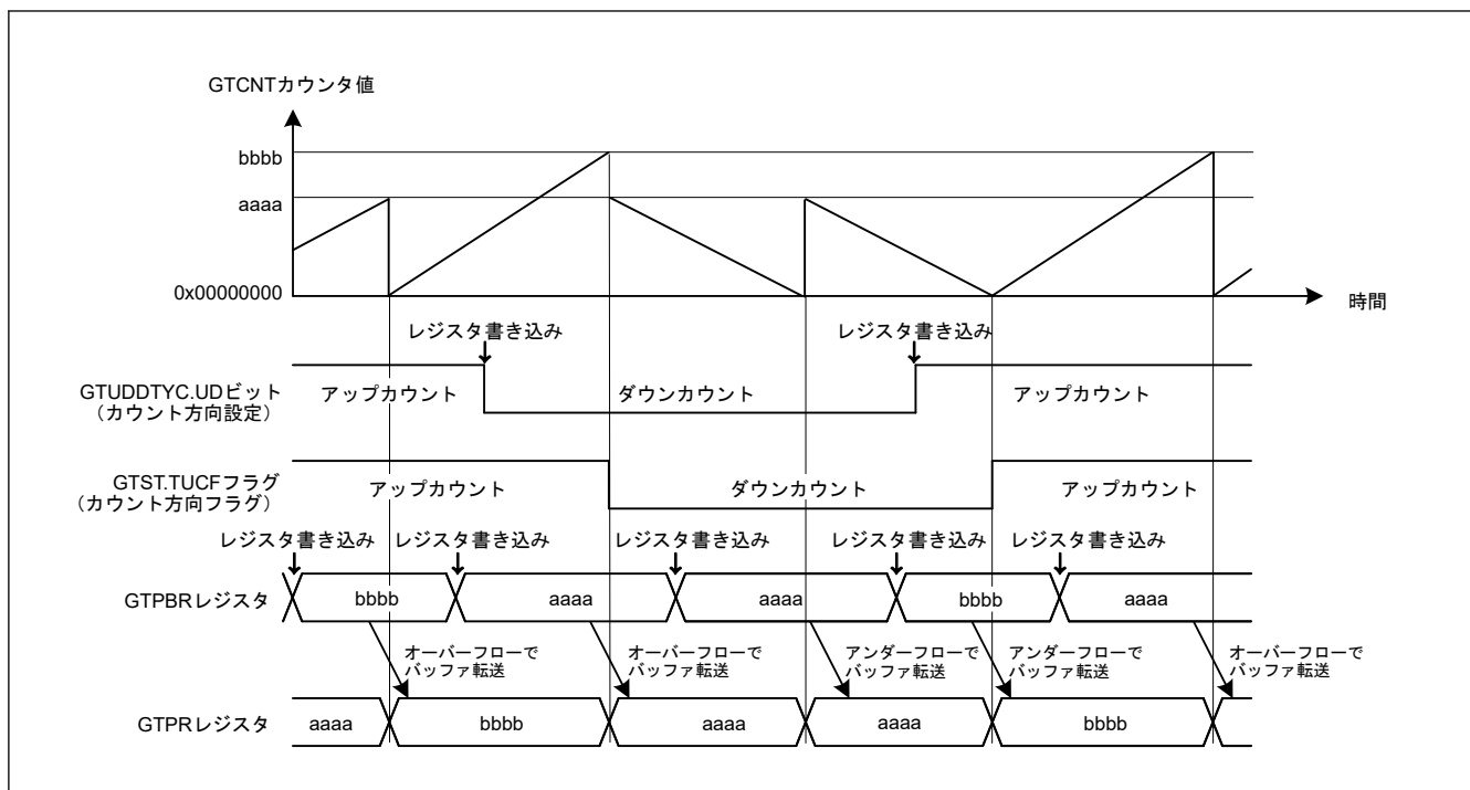
図 20.87 カウント方向切り替え機能の動作例 (バッファ動作時)
