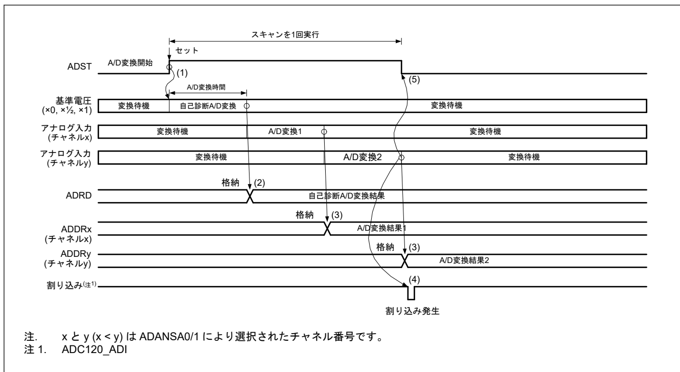
図 29.9 シングルスキャンモードの基本動作例（アナログ入力（チャンネル x と y）選択+自己診断）
