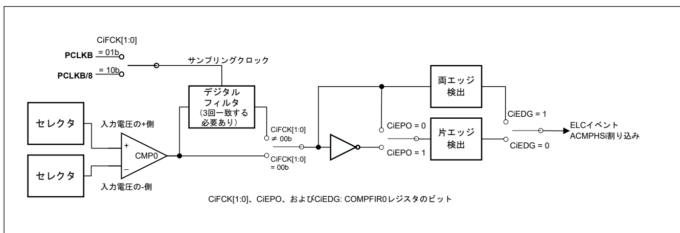
図 28.3 ノイズフィルタとエッジ検出回路の構成
