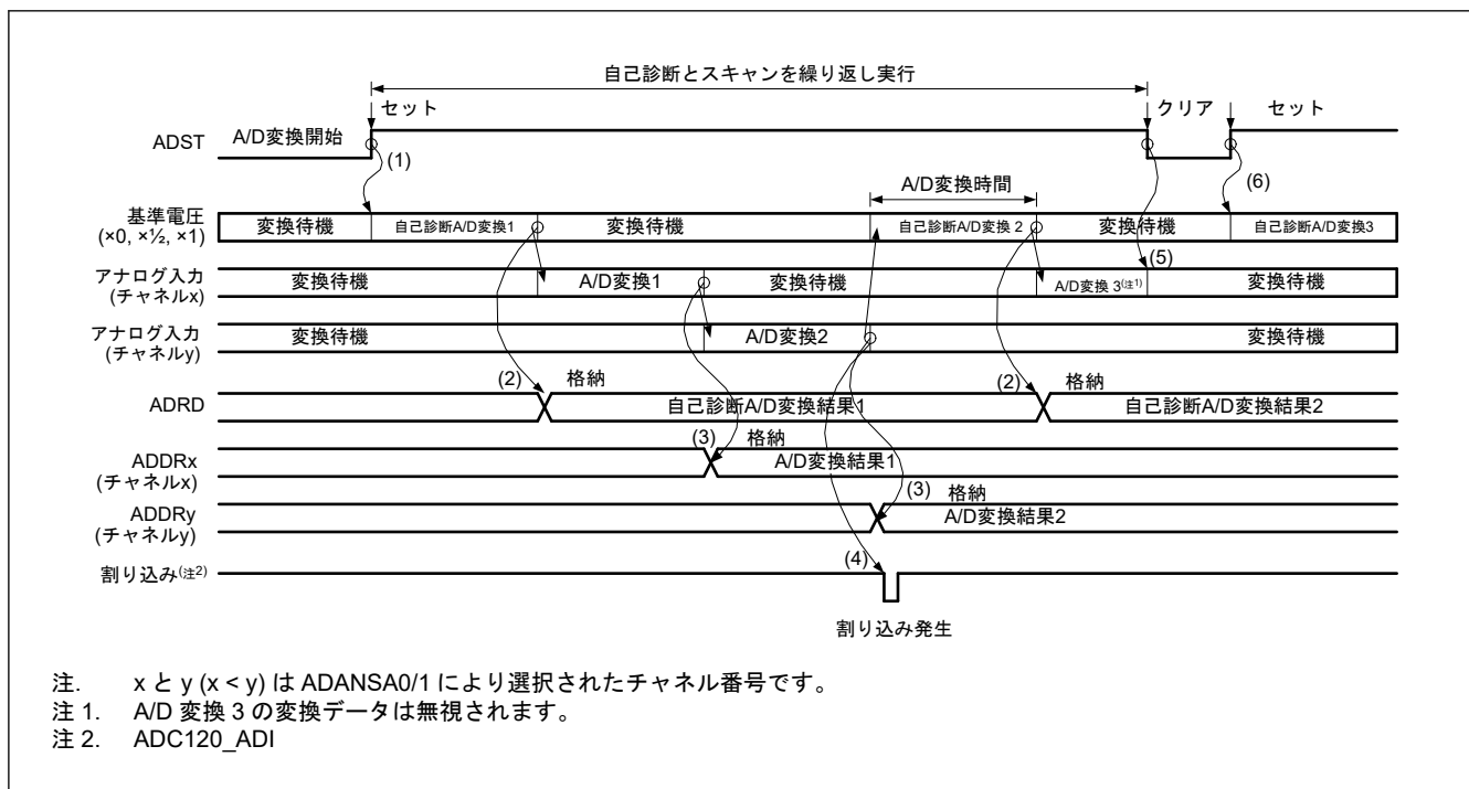
図 29.16 連続スキャンモードの基本動作例 (アナログ入力 (チャンネル x, y) 選択+自己診断)
