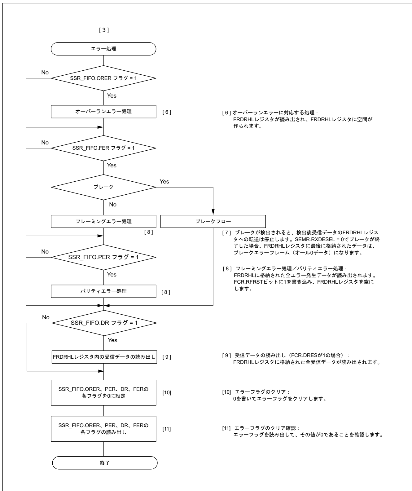
図 24.22 調歩同期式モードにおけるシリアル受信のフローチャート例（FIFO 選択、アドレス一致検出無効時）(2)
