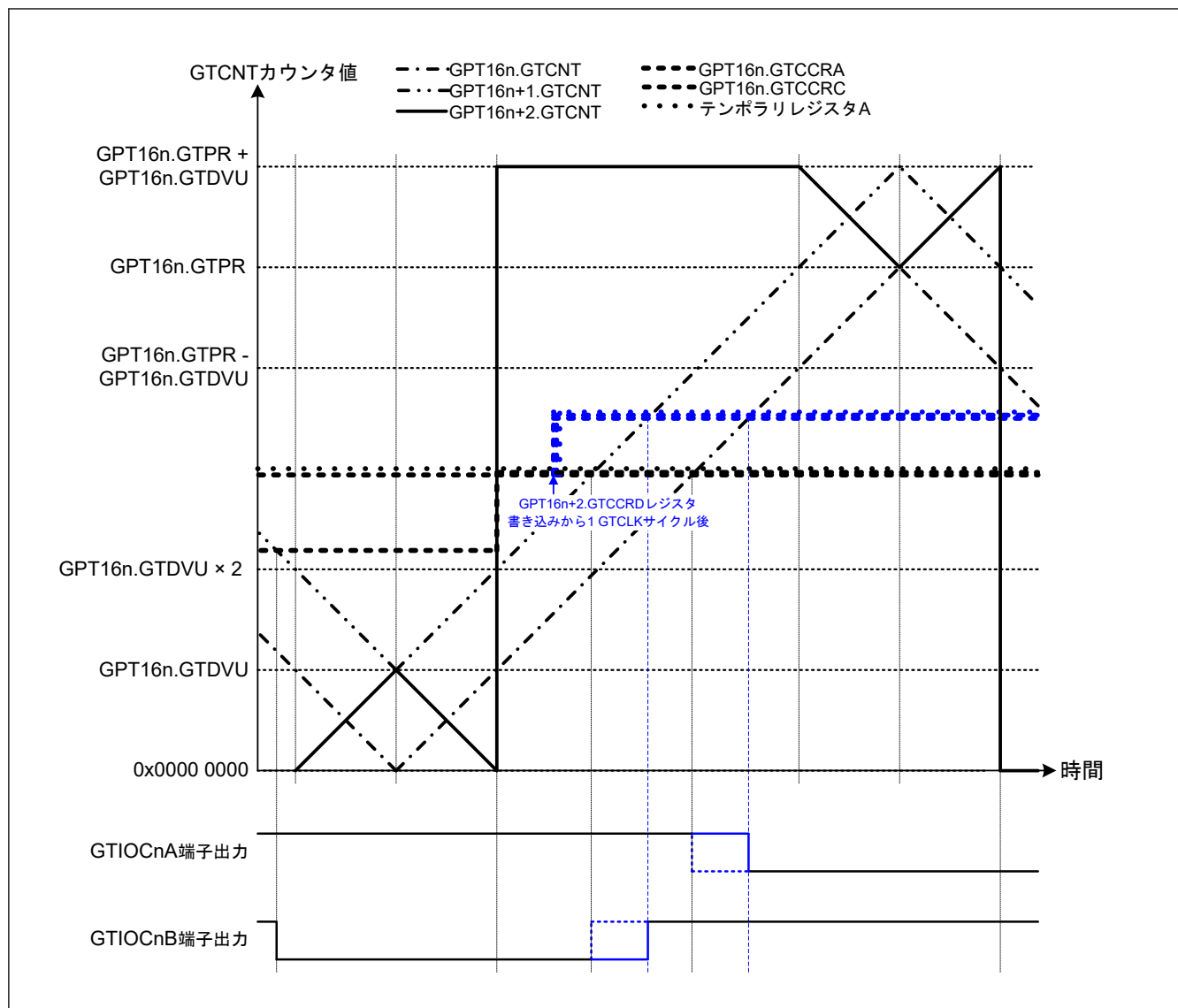
図 20.70 相補 PWM モード 4 のシングルバッファ動作例（アップカウント中間部分）（相補 PWM モード 4 のシングルバッファ動作、アップカウントの GTCCRA レジスタコンペアマッチ時：GTIOCnA 端子 = Low / GTIOCnB 端子 = High、ダウンカウントの GTCCRA レジスタコンペアマッチ時：GTIOCnA 端子 = High / GTIOCnB 端子 = Low、アップカウントのコンペアマッチ前に GPT16n+1.GTCNT 値よりも大きい値が GTCCRDR レジスタに書き込まれた場合）（n = 0）
