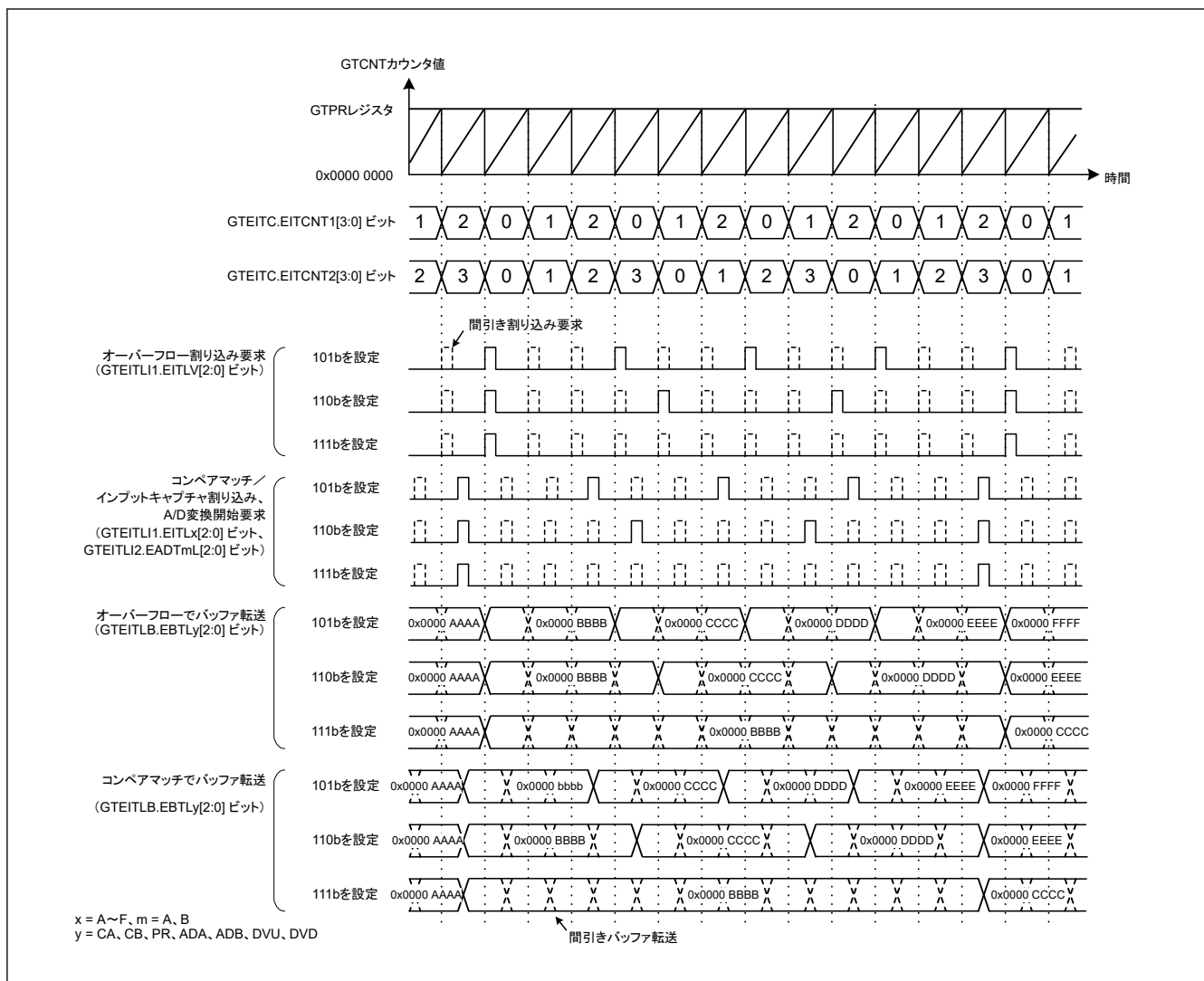
図 20.154 拡張割り込み間引き機能の動作例（三角波でアップカウント、オーバーフローのカウンタ、拡張割り込み間引き 1 間引きカウンタ：2、オーバーフローのカウンタ、拡張割り込み間引き 2 間引きカウンタ：3、拡張割り込み間引きカウンタ 2 の初期値：0、GTEITC.EITCNTk ビット (k = 1, 2) が GTEITC.EIVTTk ビット以外の期間で間引き)
