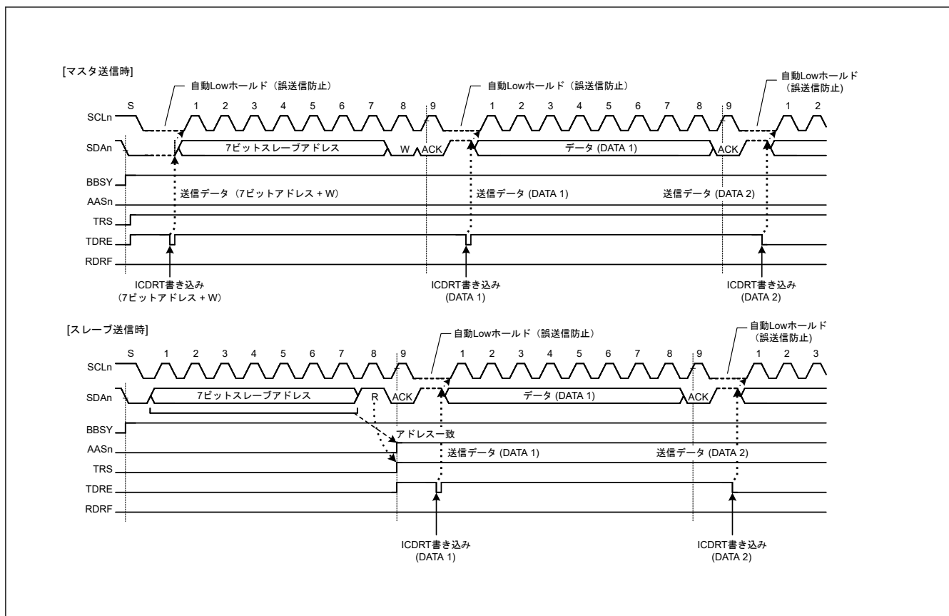
図 25.38 送信モード時の自動 Low ホールド動作
