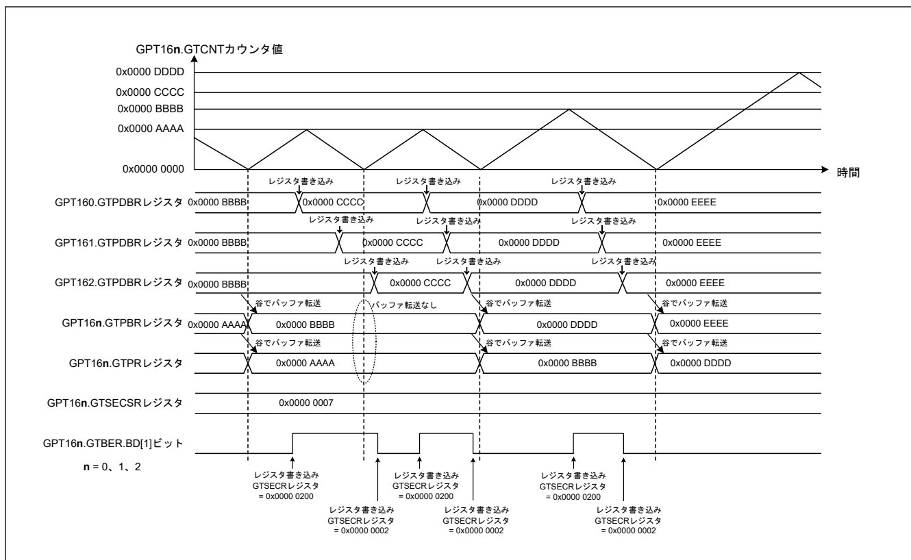
図 20.164 バッファ動作禁止の複数チャネルの動作例 (三角波、ダブルバッファ動作)
