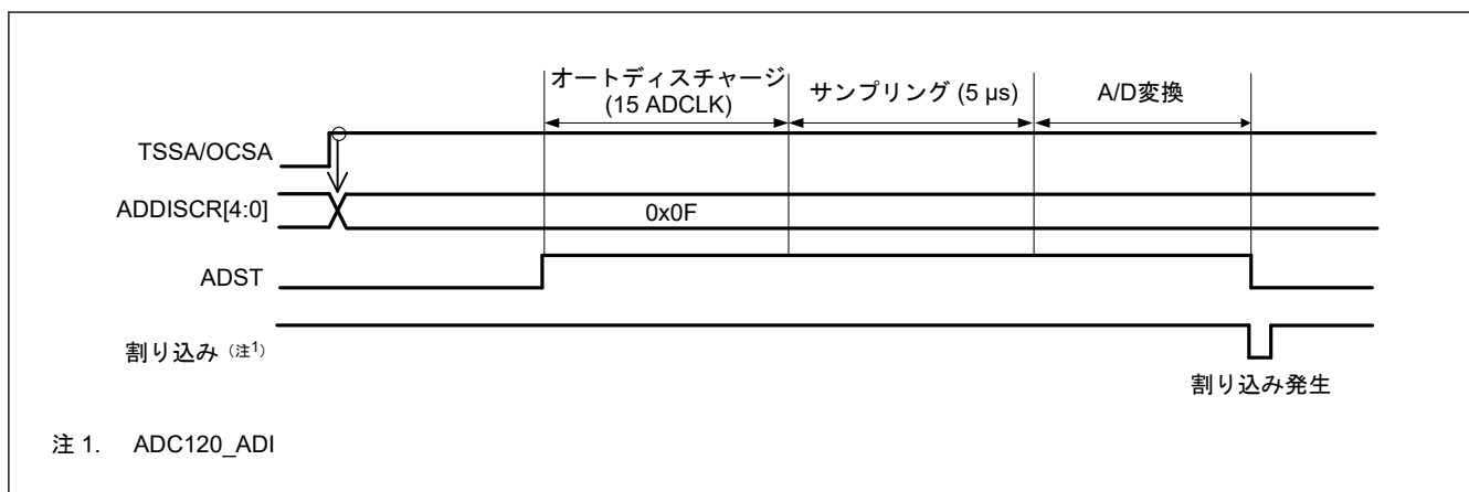
図 29.11 シングルスキャンモードの基本動作例 (温度センサ出力または内部基準電圧選択)
