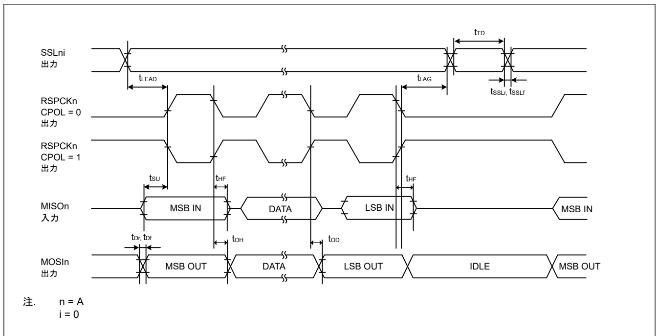
図 35.41 SPI タイミング (マスタ、CPHA = 0) (ビットレート : PCLKB を 2 分周に設定)
