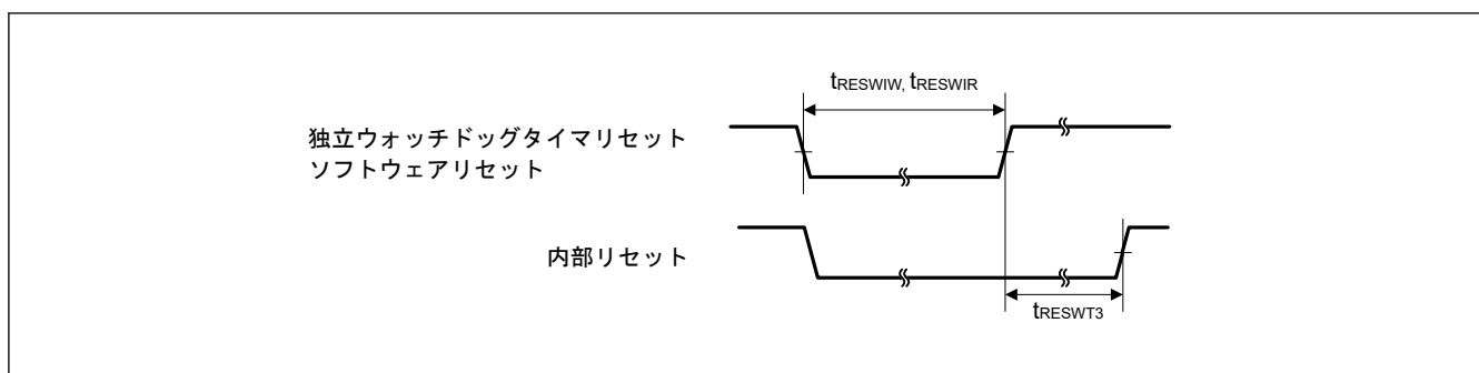
図 35.8 リセット入力タイミング (2)
