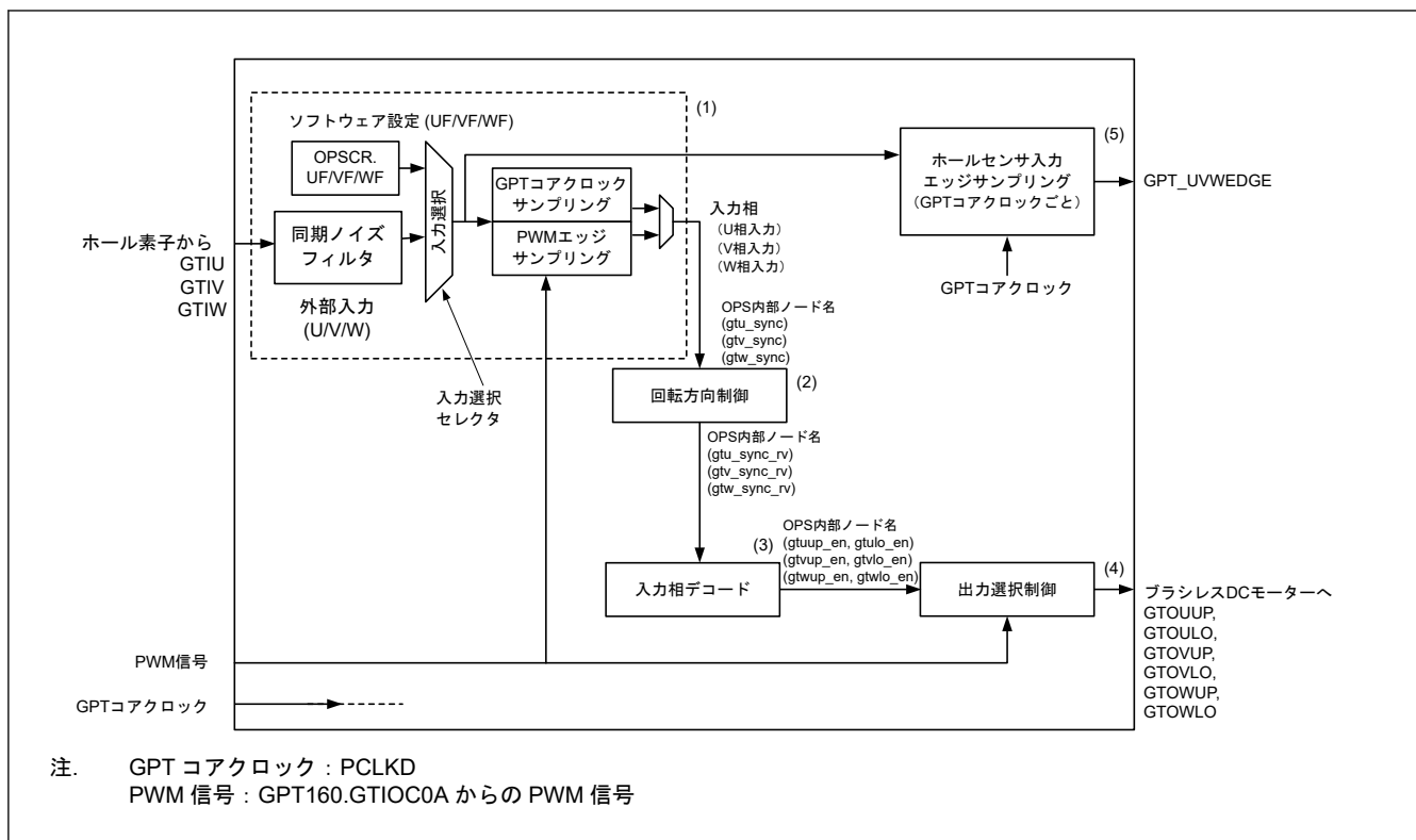
図 20.135 GPT_OPS 制御フロー概念図
