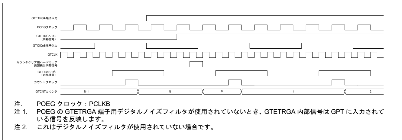
図 20.104 GTETRGA 端子入力の立ち上がりエッジに対応するカウンタクリアの動作タイミング例（ハードウェア要因によりトリガされるカウント中）
