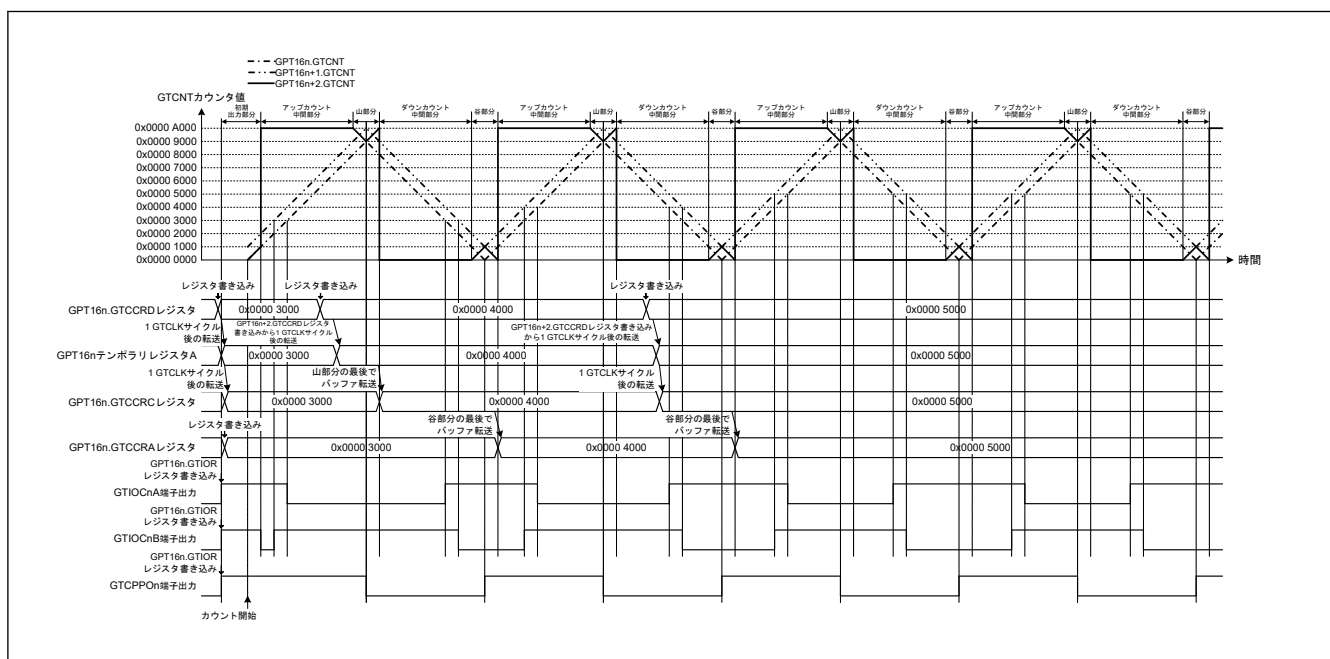
図 20.49 相補 PWM モード 2 動作例 (初期出力時 : GTIOCnA 端子 = High/GTIOCnB 端子 = High、アップカウン트의 GTCCRA レジスタコンペアマッチ時 : GTIOCnA 端子 = Low/GTIOCnB 端子 = High、ダウンカウン트의 GTCCRA レジスタコンペアマッチ時 : GTIOCnA 端子 = High/GTIOCnB 端子 = Low、デッドタイム値 : 0x0000 1000、GTCCRD レジスタを中間部分で更新) (n = 0)
