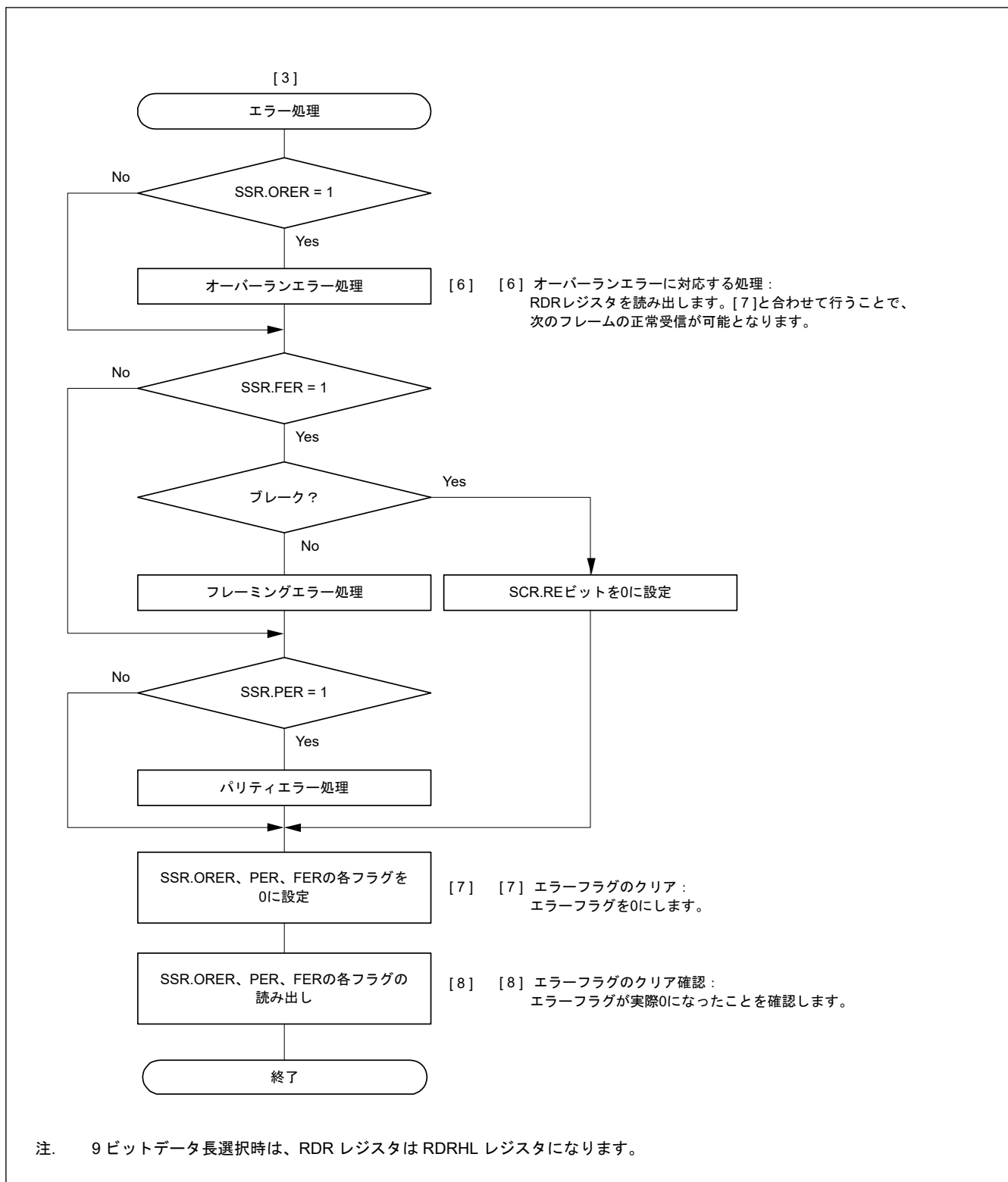
図 24.19 調歩同期式モードにおけるシリアル受信のフローチャート例（非 FIFO 選択、アドレス一致検出有効時） (3)
