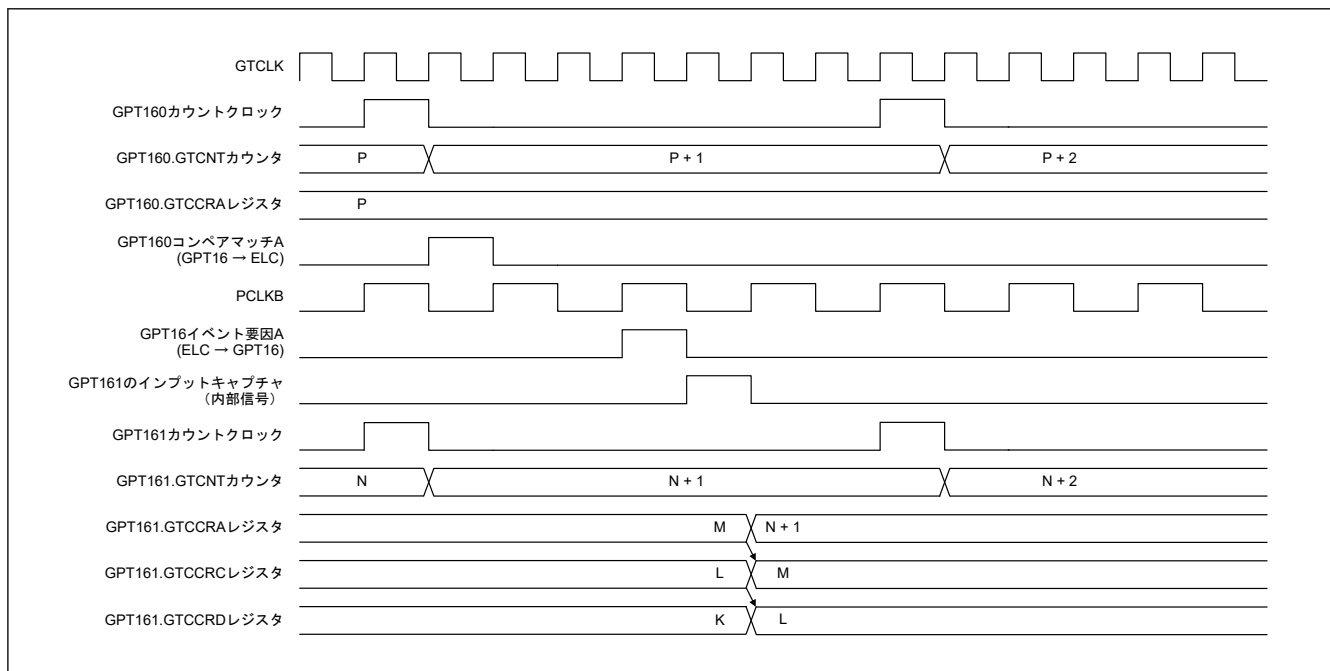
図 20.16 ELC_GPTA のイベント入力に対応するインプットキャプチャ動作のタイミング例
