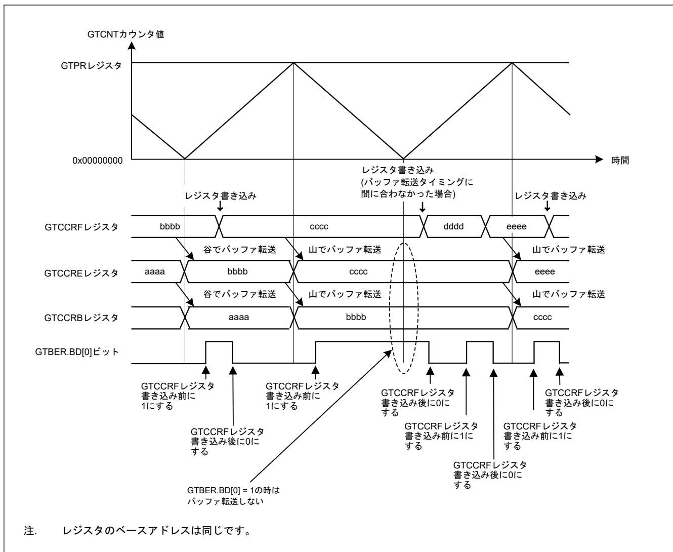
図 20.163 バッファ動作禁止の動作例（三角波、ダブルバッファ動作、谷および山の両方でバッファ転送の場合）
