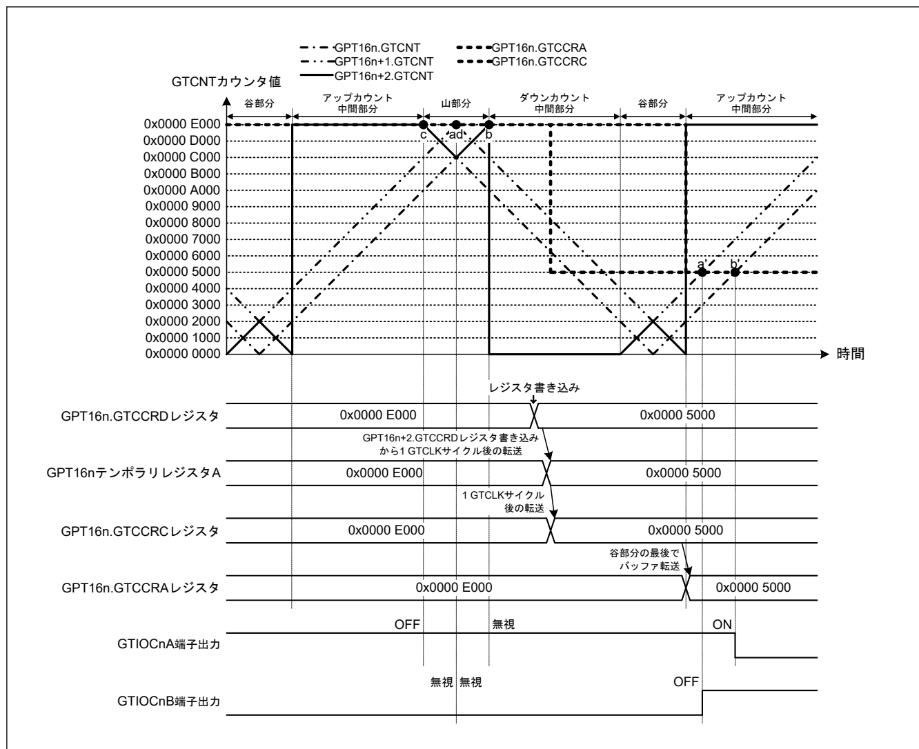
図 20.60 相補 PWM モードでのコンペアマッチ発生シーケンス動作例 (相補 PWM モード 3 シングルバッファ動作、アップカウントの GTCCRA レジスタコンペアマッチ時: GTIOcNA 端子 = Low/GTIOcNB 端子 = High、ダウンカウントの GTCCRA レジスタコンペアマッチ時: GTIOcNA 端子 = High/GTIOcNB 端子 = Low、デッドタイム値: 0x0000 2000、コンペアマッチ発生順序: c → (a, d) → b) (n = 0)
