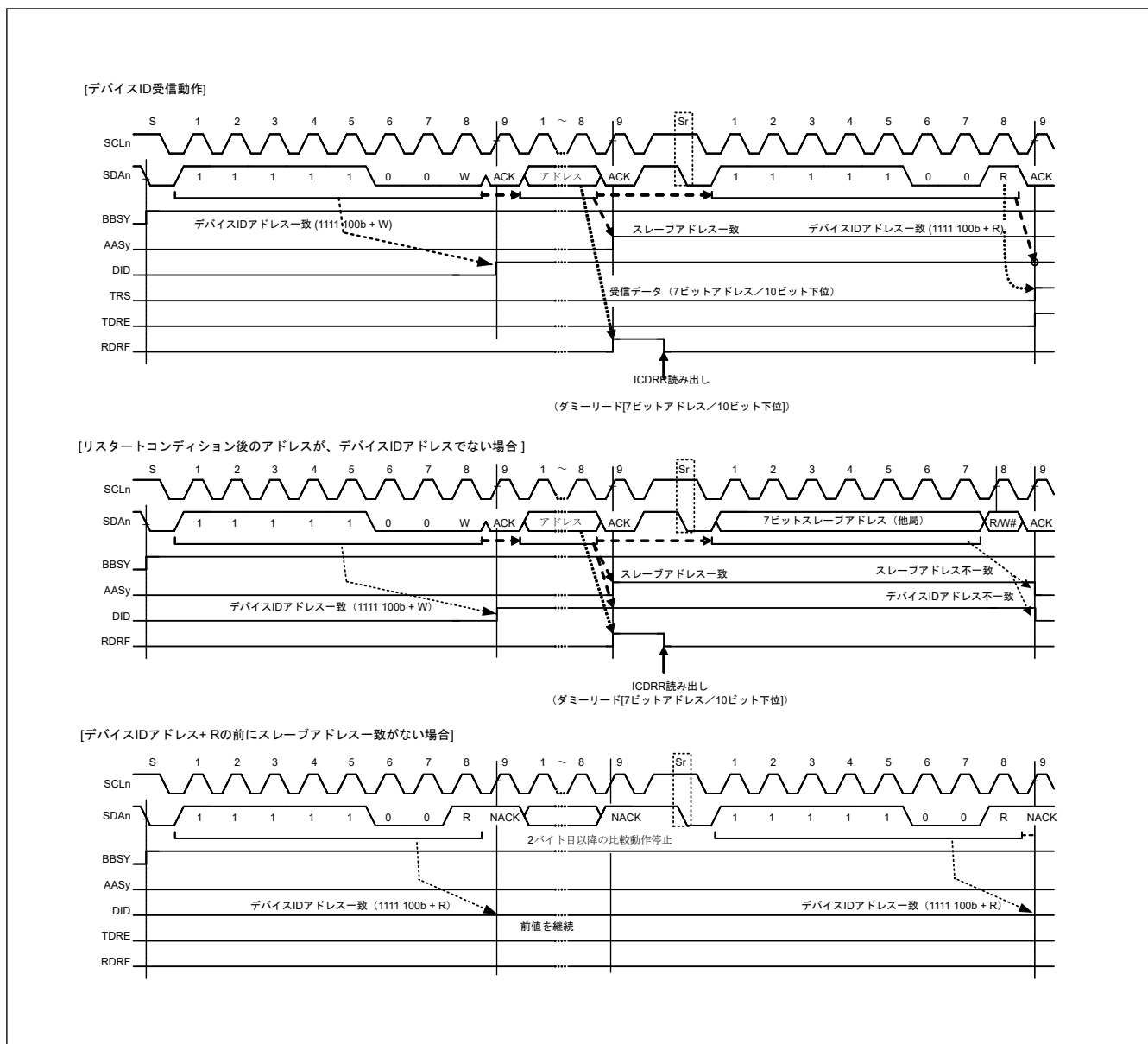
図 25.28 デバイス ID 受信時の AASn、DID フラグのセット/クリアタイミング
