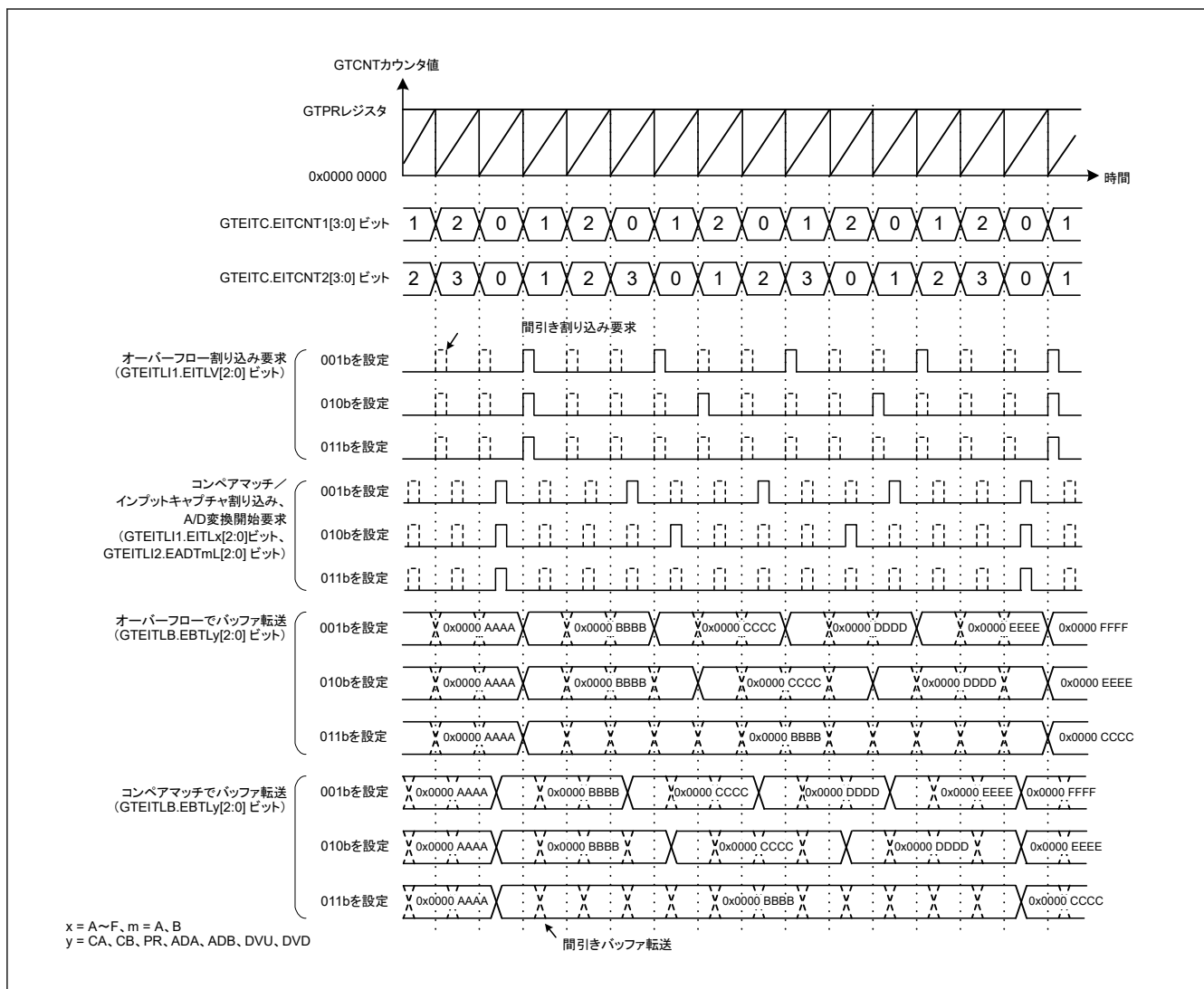
図 20.153 拡張割り込み間引き機能の動作例 (三角波でアップカウント、オーバーフローのカウンタ、拡張割り込み間引き 1 間引きカウンタ : 2、オーバーフローのカウンタ、拡張割り込み間引き 2 間引きカウンタ : 3、拡張割り込み間引きカウンタ 2 の初期値 : 0、GTEITC.EITCNTk ビット (k = 1, 2) が 0 以外の期間で間引き)
