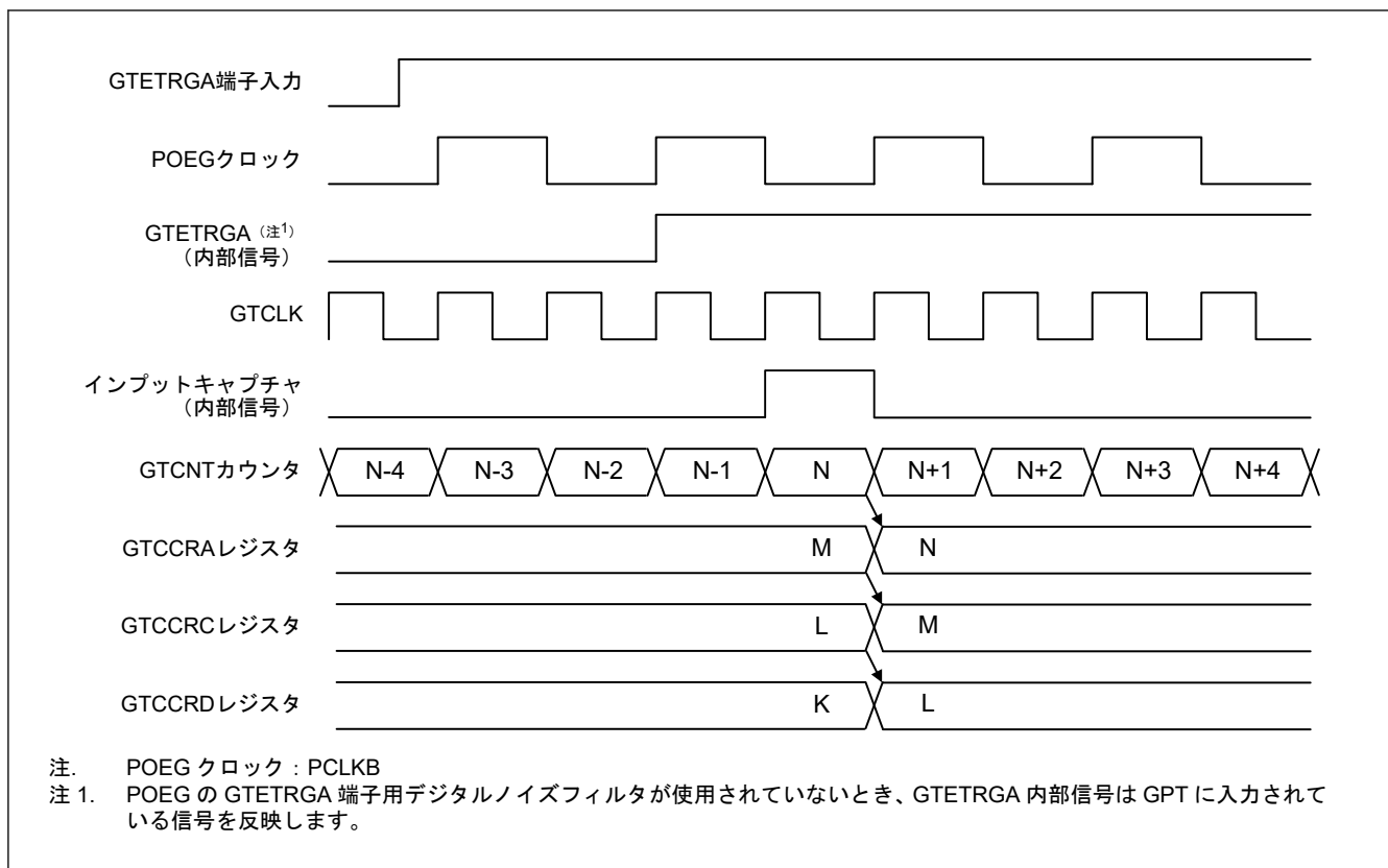
図 20.14 GTETRGA 端子の入力の立ち上がりエッジに対応するインプットキャプチャ動作のタイミング例
