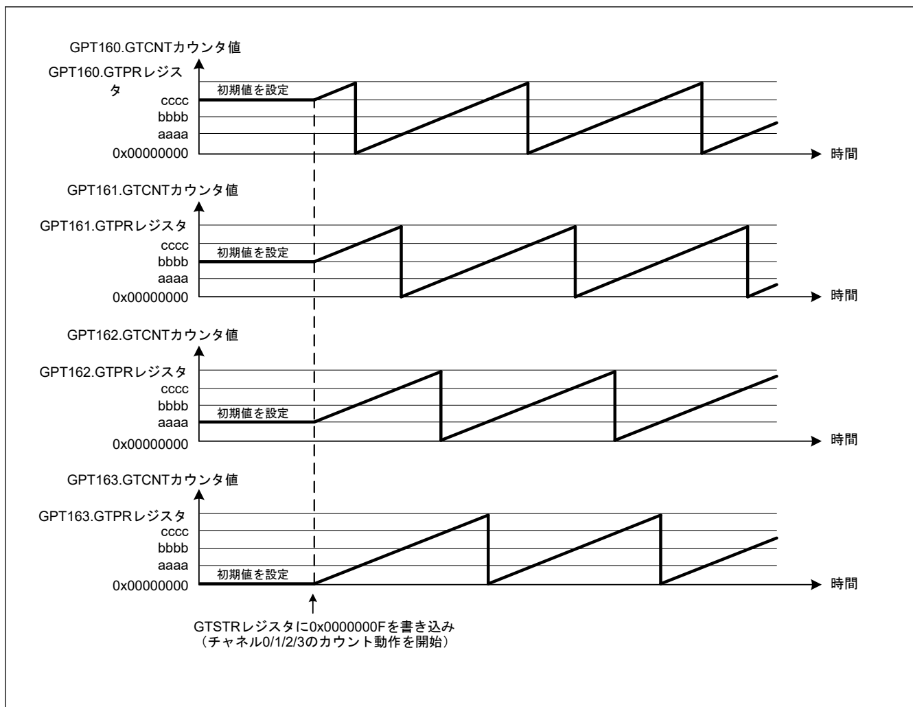
図 20.108 ソフトウェアによる位相スタート動作例 (カウント周期 (GTPR レジスタ値) が同一のとき)
