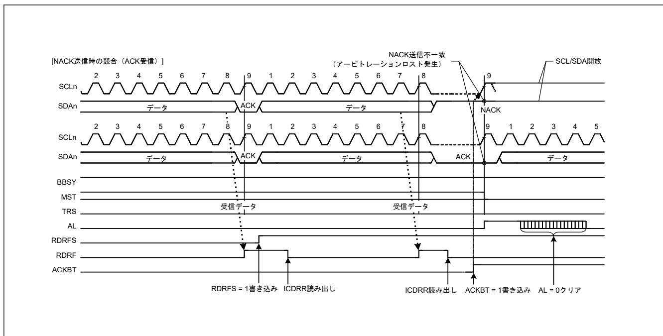
図 25.43 NACK 送信中のアービトレーションロスト検出の動作例 (NALE = 1 の場合)
