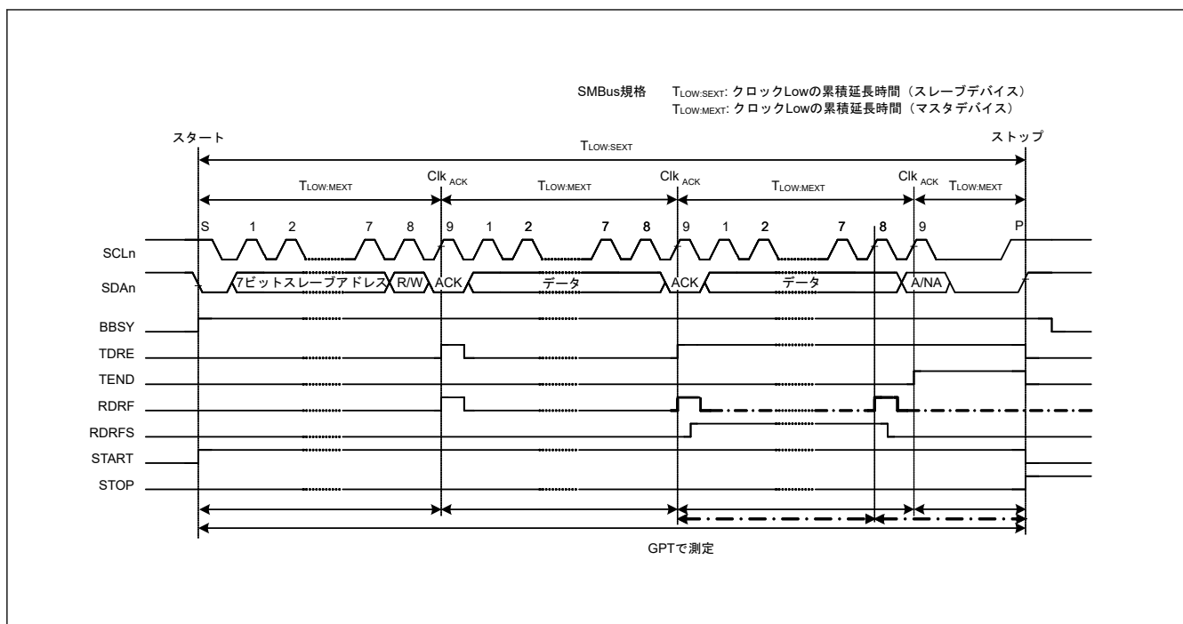
図 25.50 SMBus タイムアウト測定
