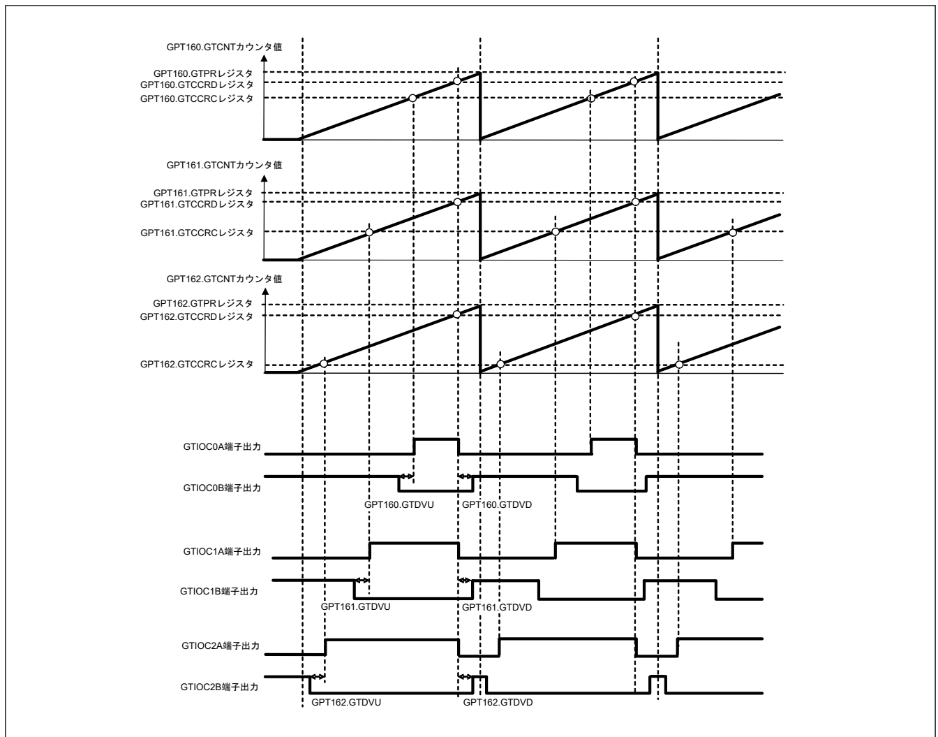
図 20.117 のこぎり波 3 相相補 PWM 出力例 (デッドタイム自動設定)
