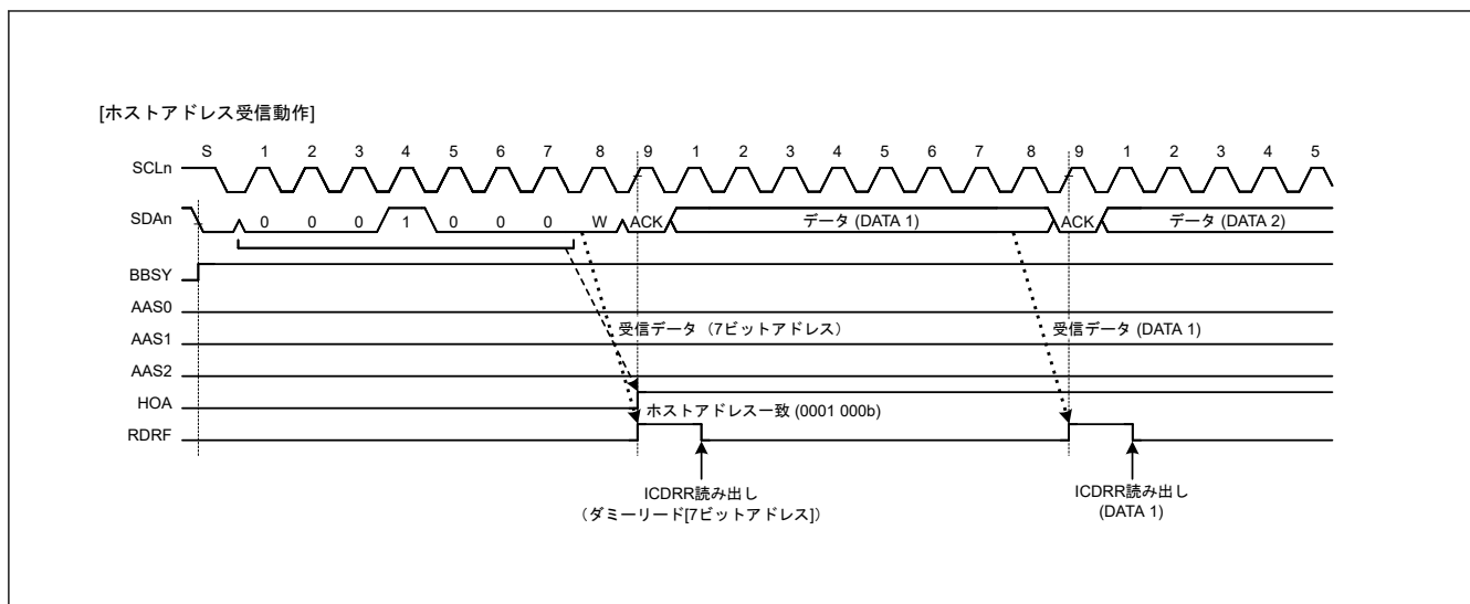
図 25.29 ホストアドレス受信時に HOA フラグが 1 になるタイミング
