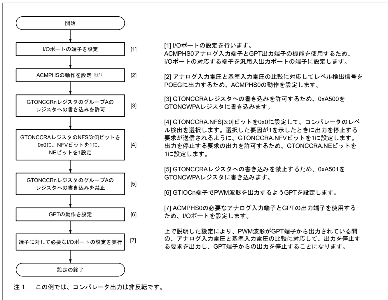
図 19.5 コンパレータによるレベル検出に対応して GTIOC 端子の出力を停止する設定の例
