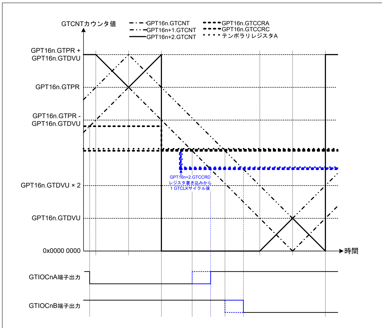
図 20.73 相補 PWM モード 4 のシングルバッファ動作の例（ダウンカウント中間部分）（相補 PWM モード 4 のシングルバッファ動作、ダウンカウントの GTCCRA レジスタコンペアマッチ時：GTIOCnA 端子 = Low / GTIOCnB 端子 = High、ダウンカウントの GTCCRA レジスタコンペアマッチ時：GTIOCnA 端子 = High / GTIOCnB 端子 = Low、ダウンカウントのコンペアマッチ前に GPT16n.GTCNT 値よりも小さい値が GTCCRD レジスタに書き込まれた場合）（n = 0）
