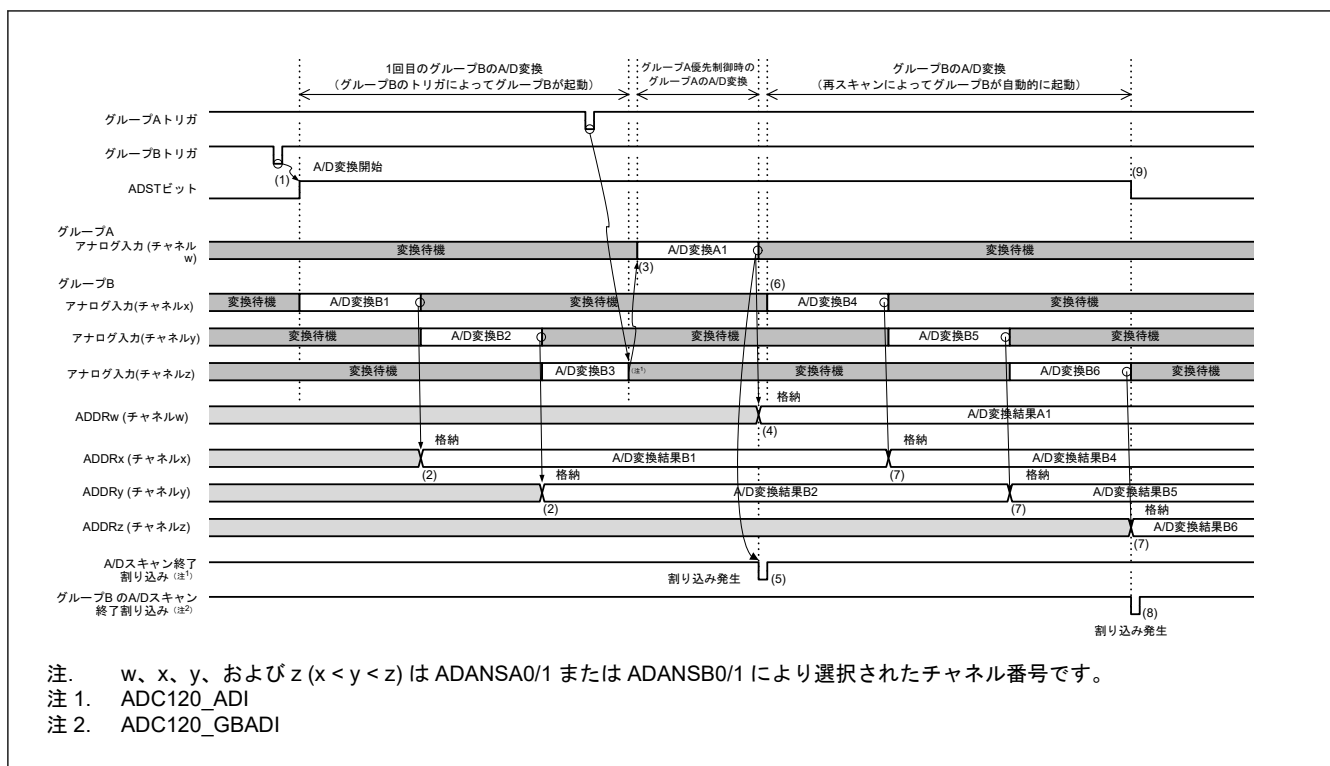
図 29.21 グループ優先動作の例 1-1: グループ B スキャン中のグループ A トリガ入力、再スキャンあり (ADGSPCR.GBRSCN = 1、ADGSPCR.GBRP = 0 の場合)
