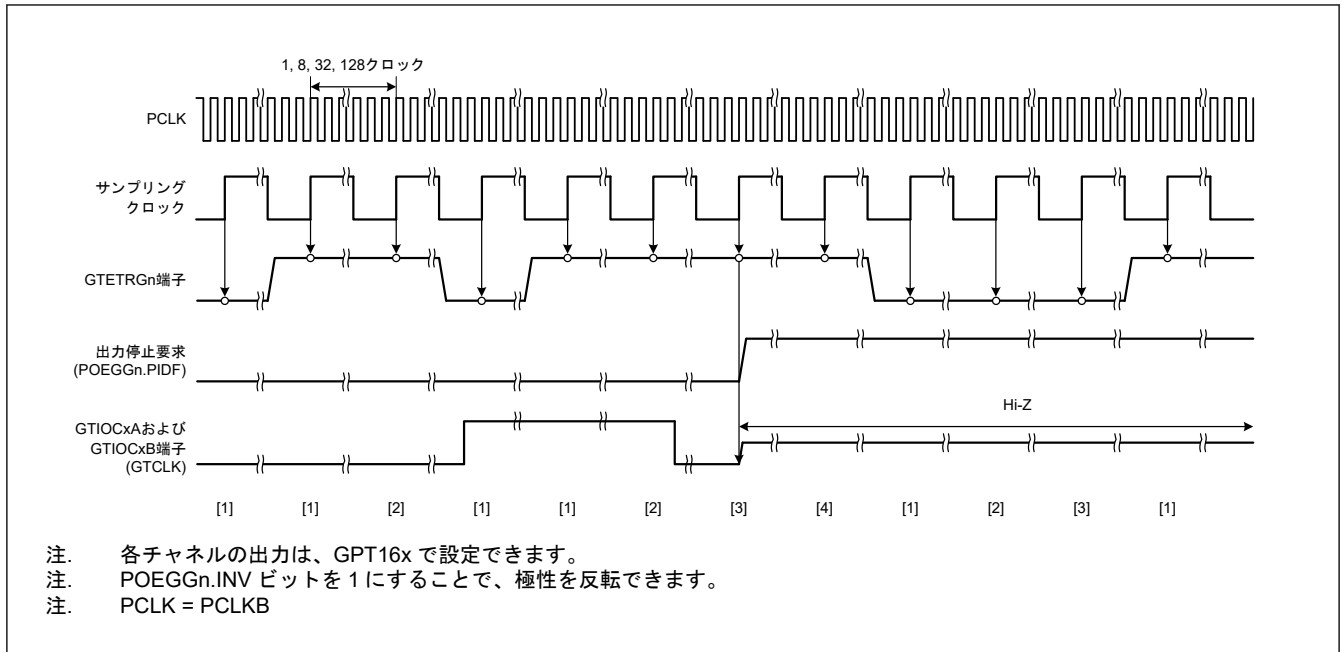
図 19.2 デジタルノイズフィルタの動作例
