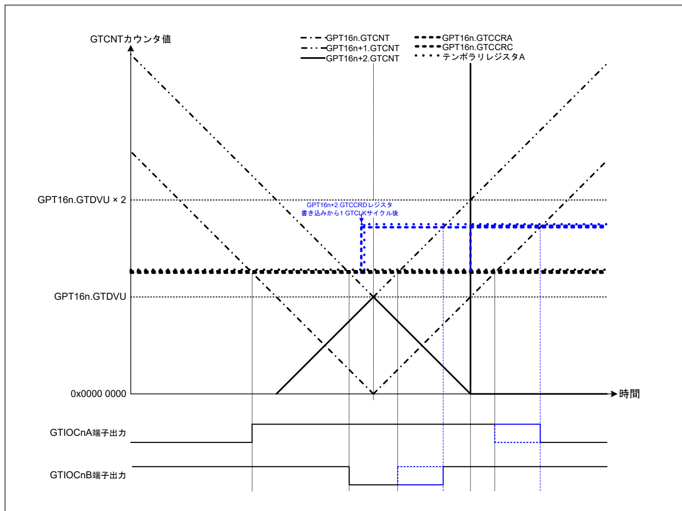
図 20.74 相補 PWM モード 4 のシングルバッファ動作例（ダウンカウント谷部分）（相補 PWM モード 4 のシングルバッファ動作、アップカウントの GTCCRA レジスタコンペアマッチ時：GTIOcNA 端子 = Low / GTIOcNB 端子 = High、ダウンカウントの GTCCRA レジスタコンペアマッチ時：GTIOcNA 端子 = High / GTIOcNB 端子 = Low、ダウンカウントのコンペアマッチ後に GPT16n+2.GTCNT 値よりも大きい値が GTCCRD レジスタに書き込まれた場合）（ n = 0 ）
