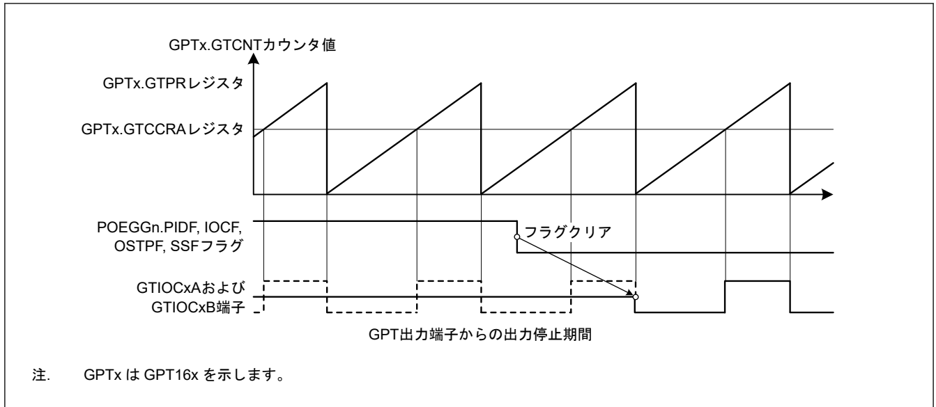
図 19.3 出力停止要求の解除後に GPT 出力端子からの出力を再度有効化するタイミング
