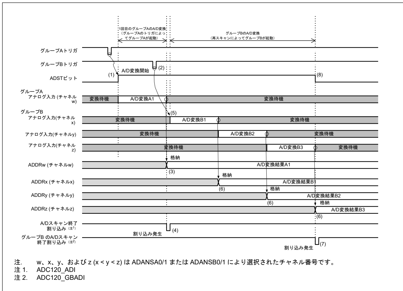
図 29.23 グループ優先動作の例 1-3 : グループ A スキャン中のグループ B トリガ入力、再スキャンあり (ADGSPCR.GBRSCN = 1、ADGSPCR.GBRP = 0 の場合)
