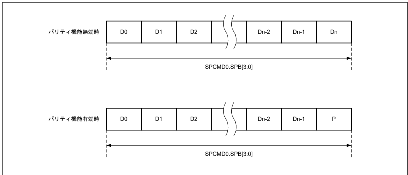
図 26.12 パリティ機能無効時と有効時のデータフォーマット
