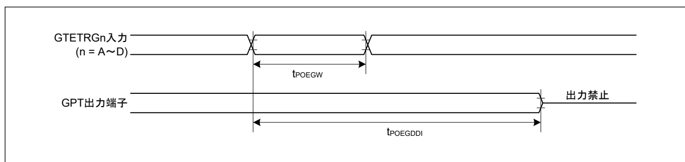
図 35.20 GTETRn 端子の入力レベル検出に直接対応した POEG の出力禁止時間
