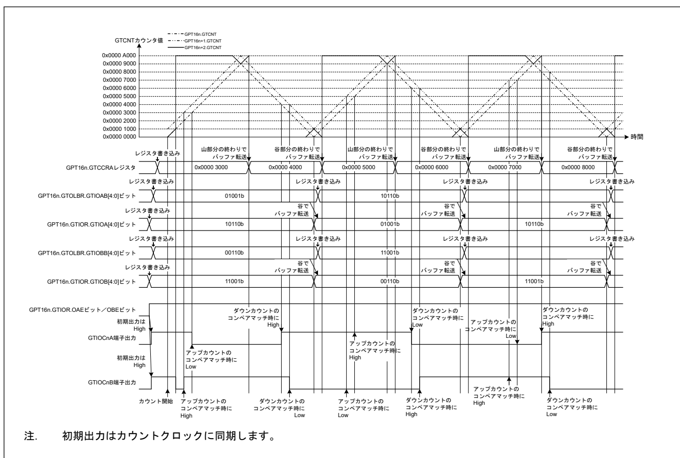
図 20.37 GTIOA ビットおよび GTIOB ビットのバッファ操作例 (相補 PWM モード 3、谷でバッファ転送)
