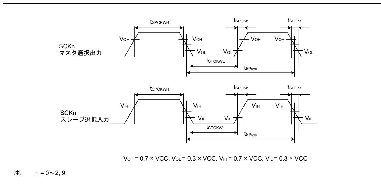
図 35.33 SCI 簡易 SPI モードクロックタイミング
