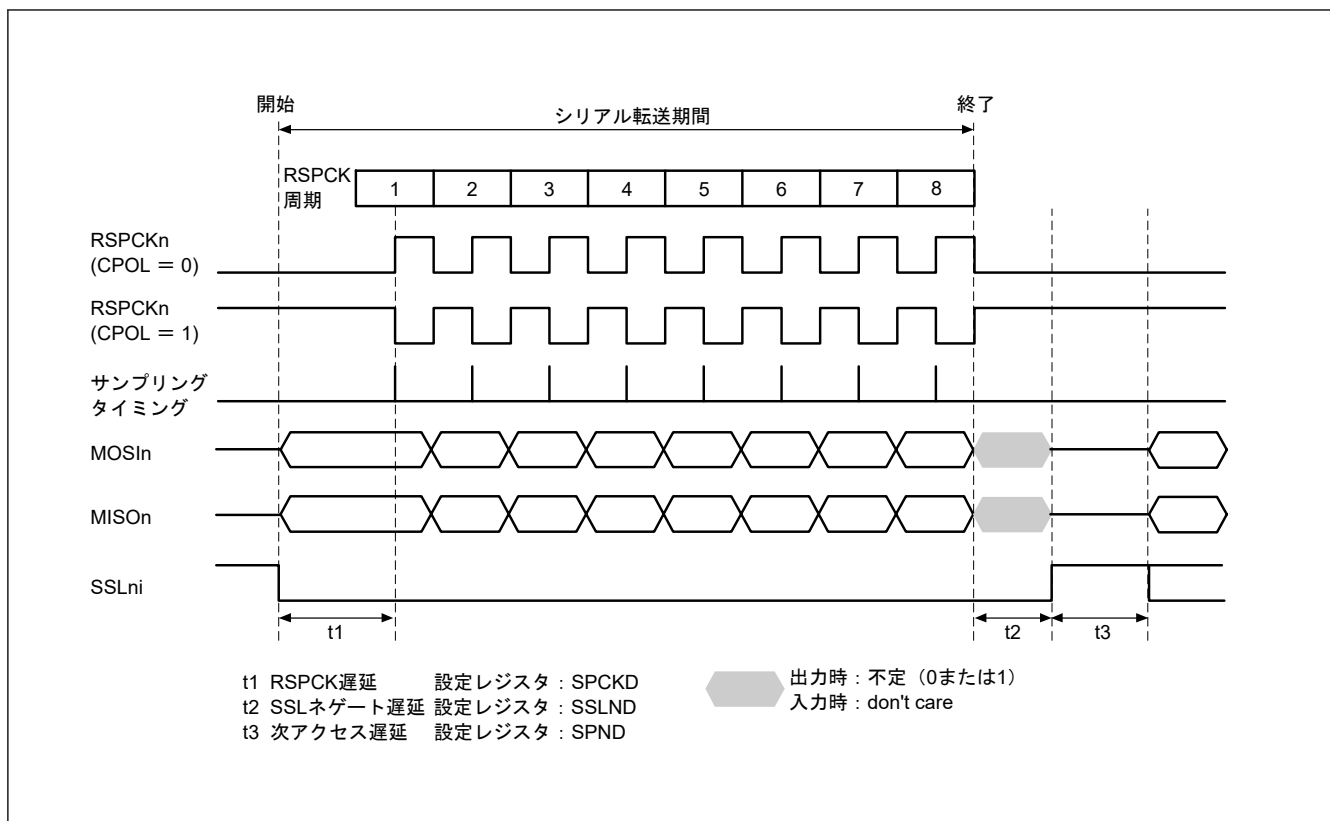
図 26.21 SPI 転送フォーマット (CPHA = 0 の場合)
