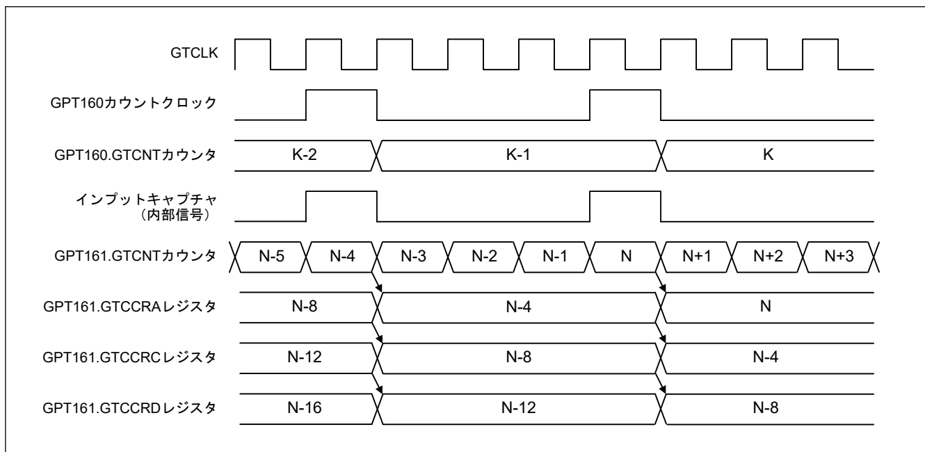
図 20.17 他のチャンネルからのカウントクロックに対応するインプットキャプチャ動作のタイミング例
