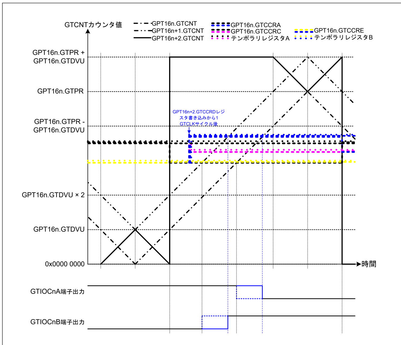
図 20.75 相補 PWM モード 4 のダブルバッファ動作例（アップカウント中間部分）（相補 PWM モード 4 のダブルバッファ動作、アップカウントの GTCCRA レジスタコンペアマッチ時：GTIOcNA 端子 = Low / GTIOcNB 端子 = High、ダウンカウントの GTCCRA レジスタコンペアマッチ時：GTIOcNA 端子 = High / GTIOcNB 端子 = Low、アップカウントのコンペアマッチ前に GPT16n+1.GTCNT 値よりも大きい値が GTCCRF レジスタに書き込まれた場合）（n = 0）
