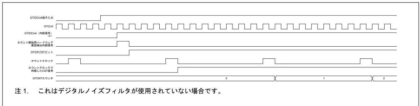
図 20.91 GTIOcNA 端子の入力の立ち上がりエッジに対応するカウントスタート動作のタイミング例
