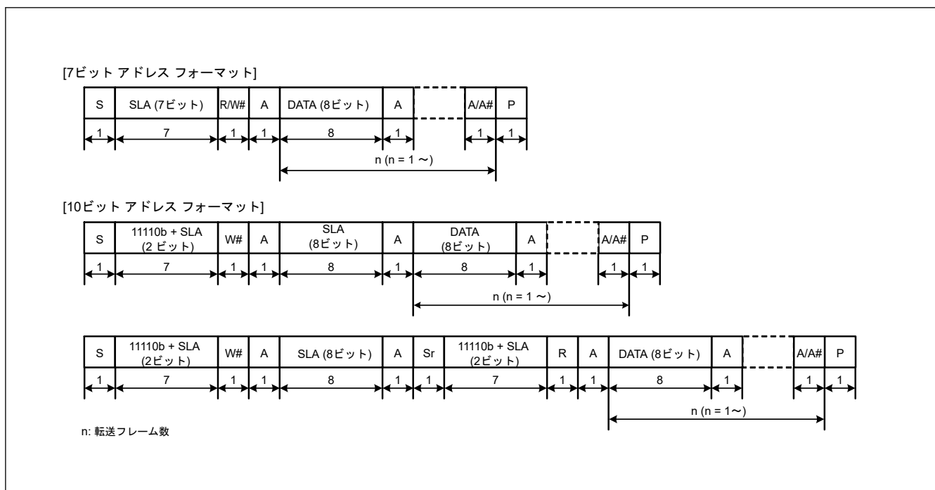
図 25.3 I 2 C バスフォーマット
