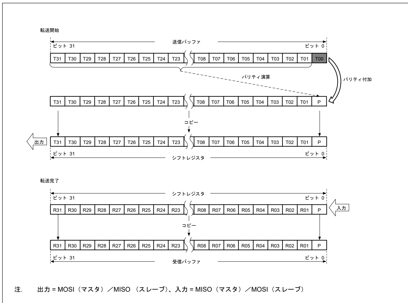
図 26.17 MSB ファースト転送 (32 ビットデータ/パリティ機能有効)
