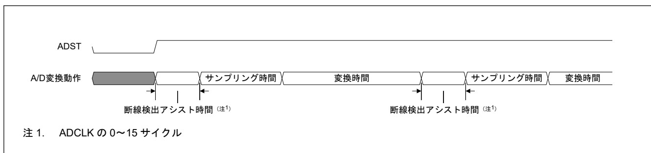
図 29.31 断線検出アシスト機能を使用した場合の A/D 変換動作図
