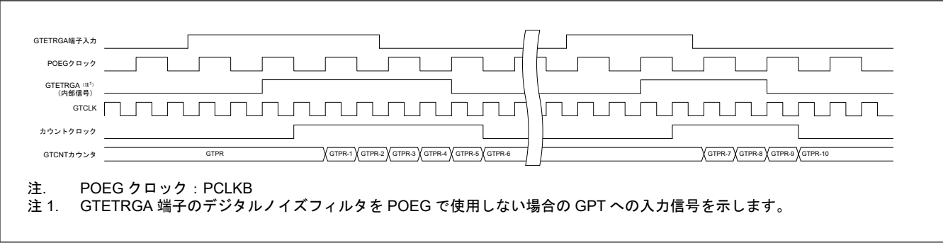
図 20.134 外部パルス幅測定機能の例（ダウンカウント）
