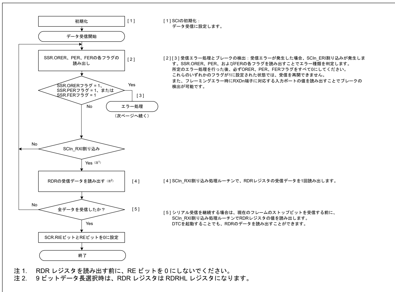
図 24.15 調歩同期式モードにおけるシリアル受信のフローチャート例（非 FIFO 選択、アドレス一致検出無効時） (1)
