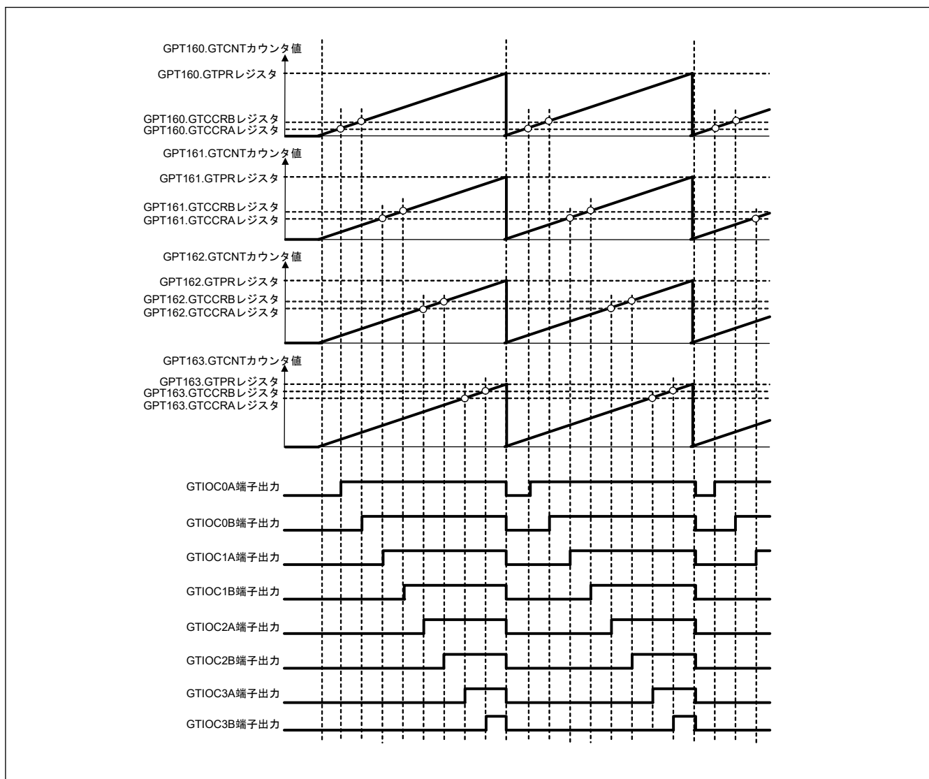
図 20.115 同期 PWM 出力例
