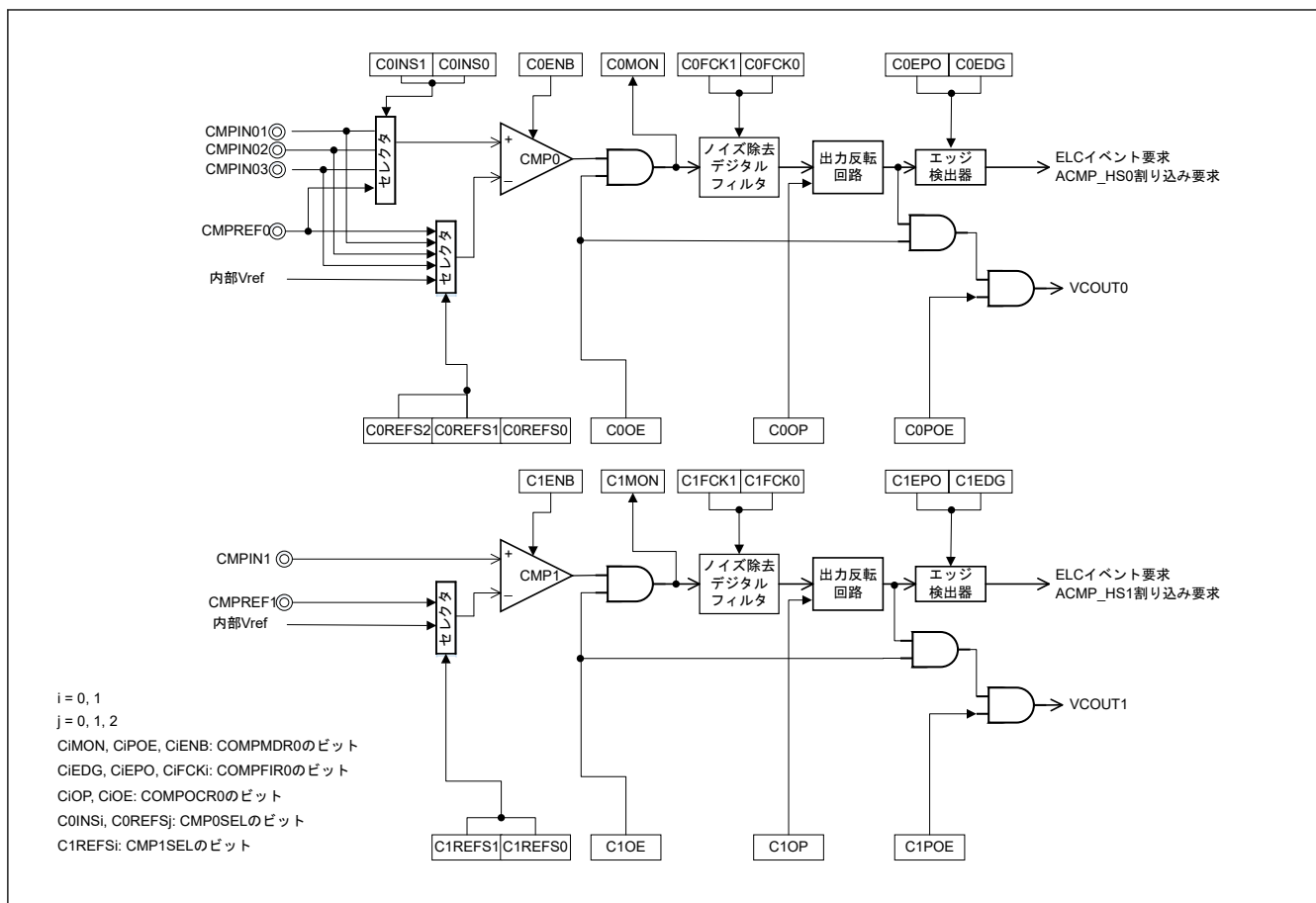
図 28.1 ACMPHS ブロック図
