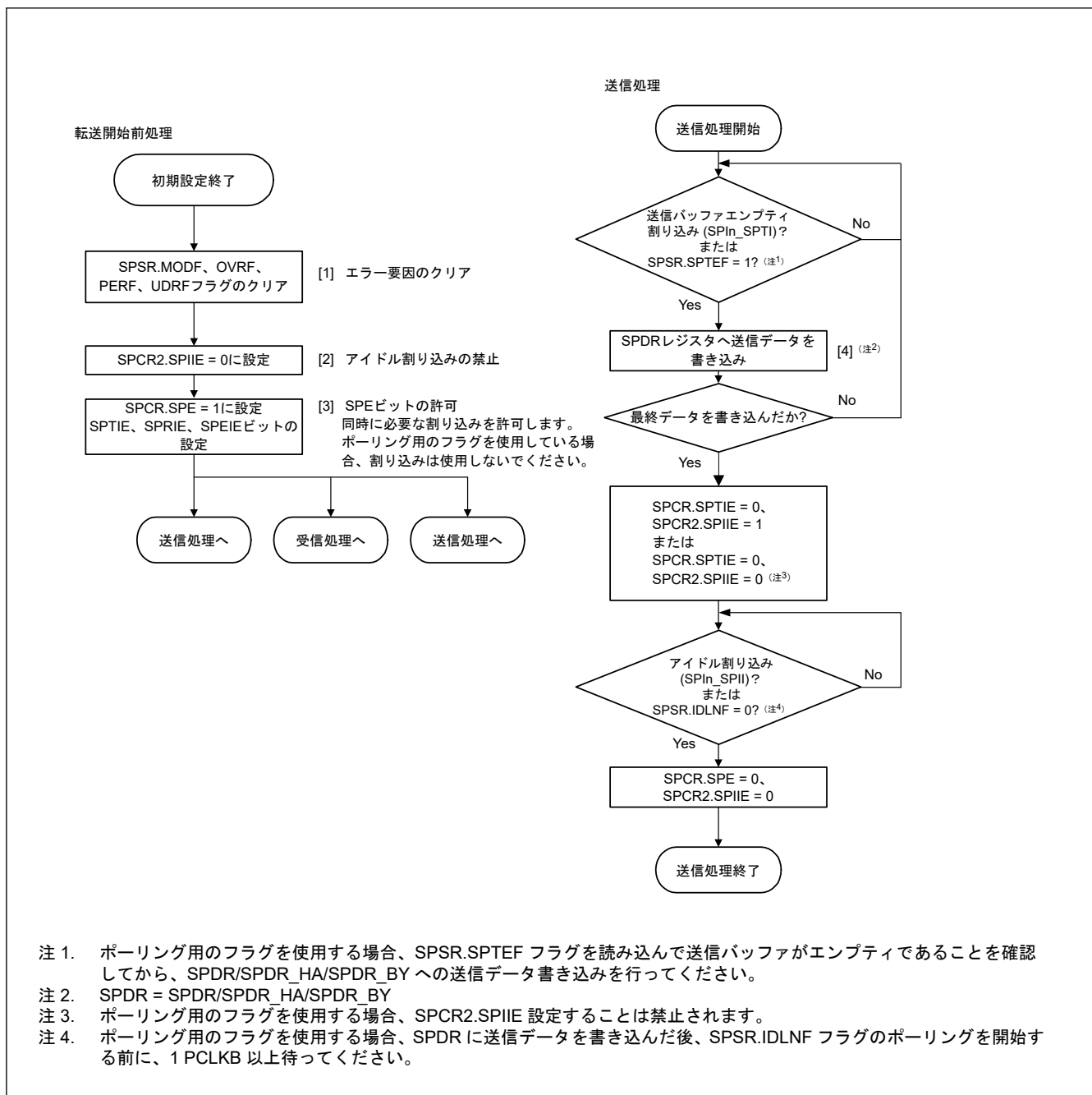
図 26.32 マスタモードでの送信フロー
