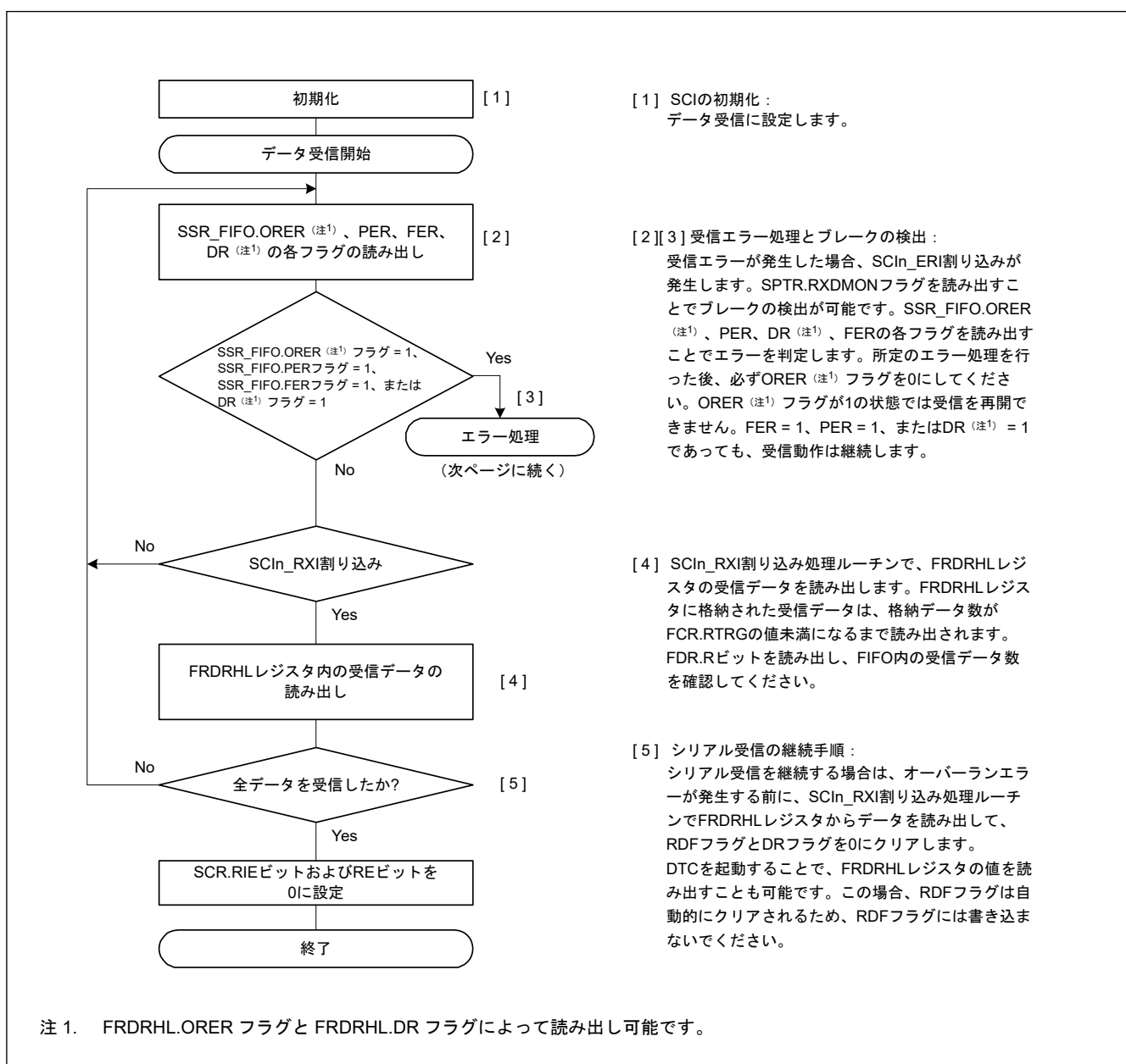
図 24.21 調歩同期式モードにおけるシリアル受信のフローチャート例 (FIFO 選択、アドレス一致検出有効時) (1)
