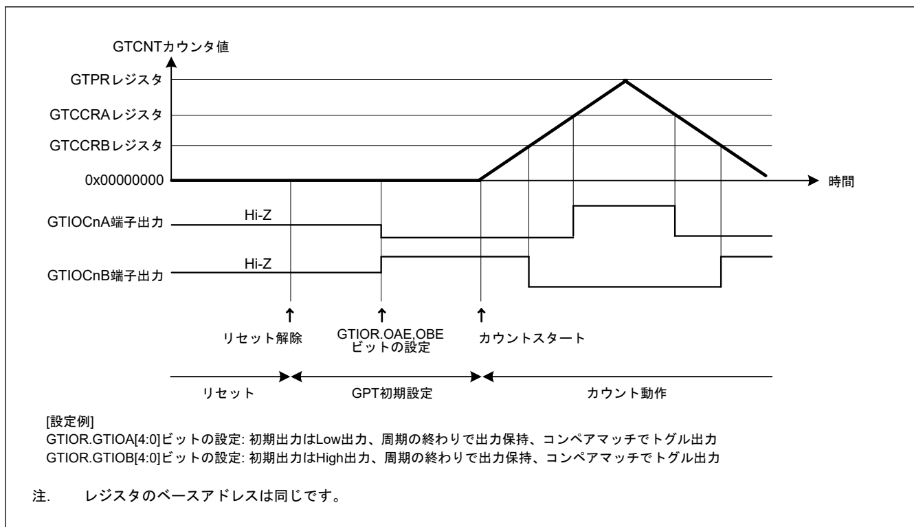
図 20.181 リセット後の端子設定例
