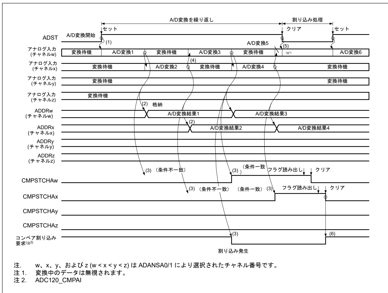
図 29.26 コンペア機能の動作例 (アナログ入力 (チャンネル w~z) を比較)
