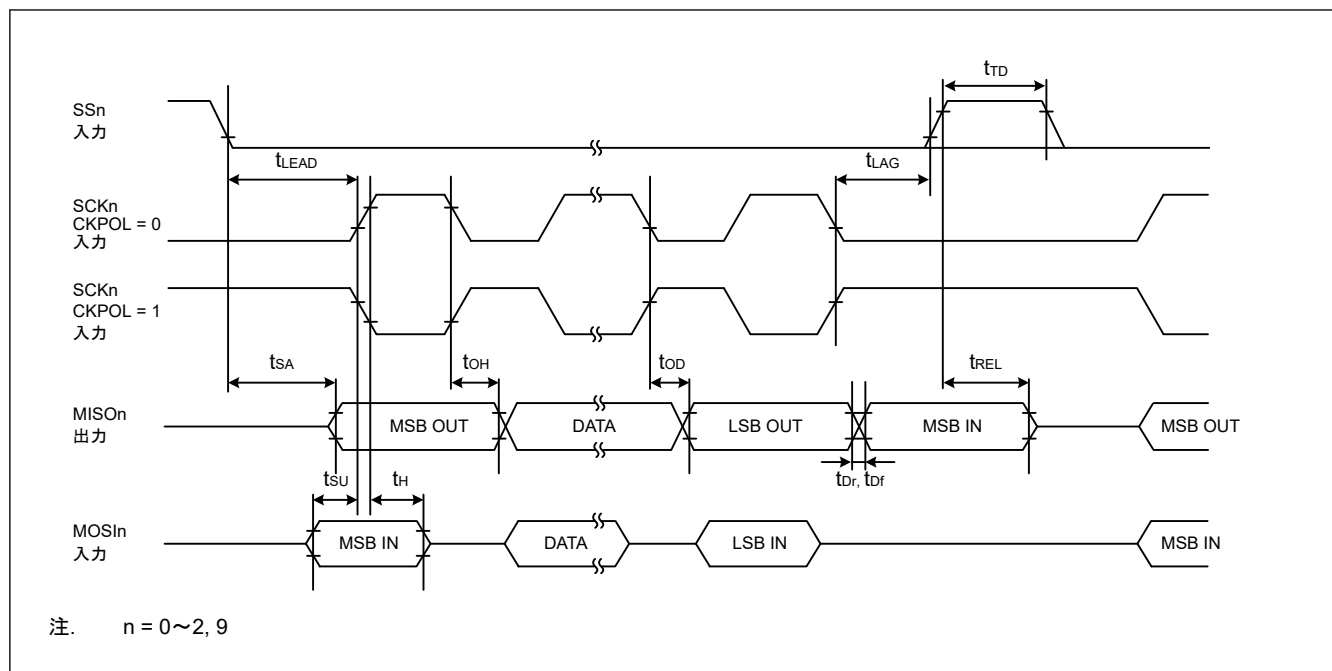
図 35.36 SCI 簡易 SPI モードタイミング (スレーブ、CKPH = 1)
