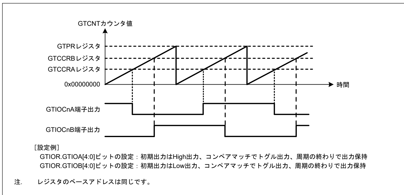
図 20.11 トグル出力動作例 (1)
