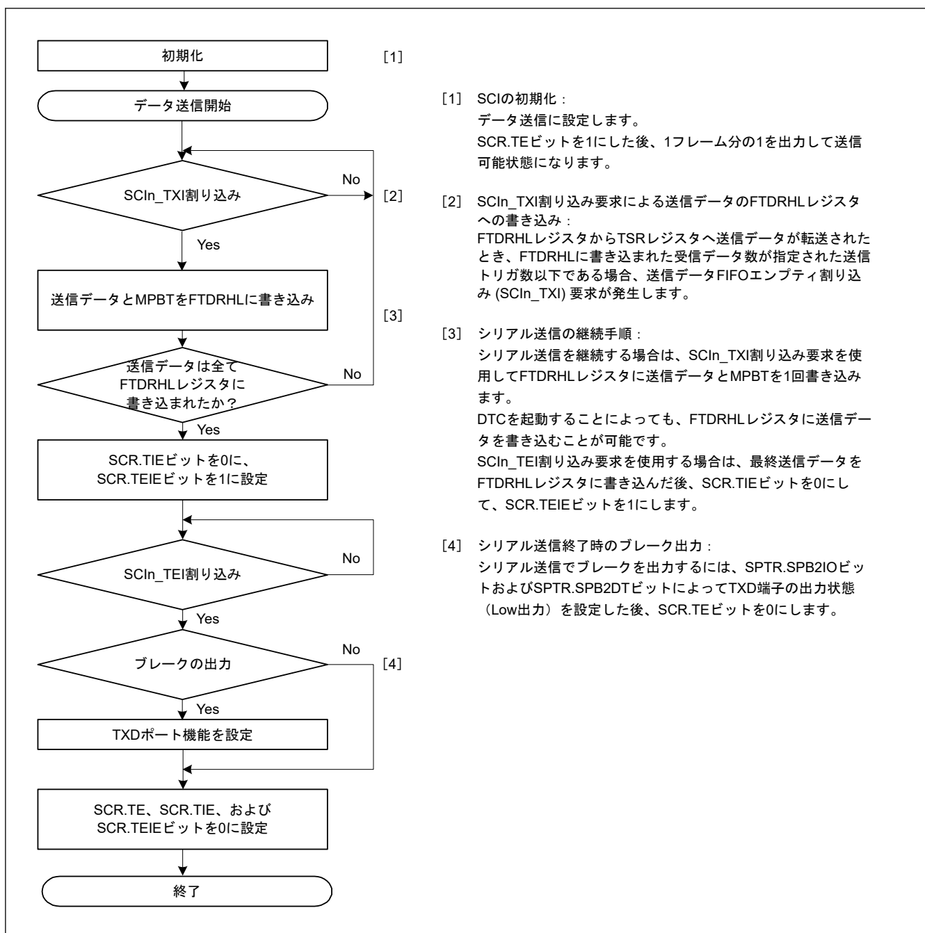
図 24.29 マルチプロセッサモードにおけるシリアル送信のフローチャート例 (FIFO 選択時)
