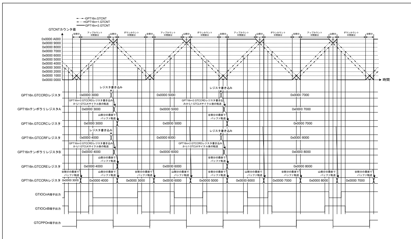
図 20.54 相補 PWM モード 3 動作例 (ダブルバッファ動作、アップカウントの GTCCRA レジスタコンペアマッチ時 : GTIOChA 端子 = Low/GTIOChB 端子 = High、ダウンカウントの GTCCRA レジスタコンペアマッチ時 : GTIOChA 端子 = High/GTIOChB 端子 = Low、デッドタイム値 : 0x0000 1000、GTCCRD レジスタを山部分と谷部分で更新) (n = 0)
