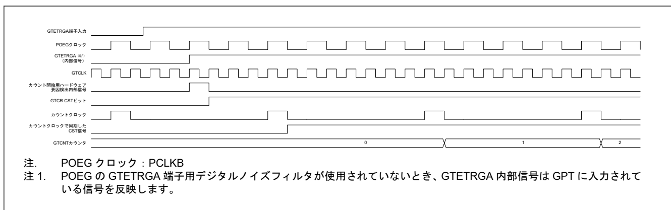
図 20.90 GTETRGA 端子の入力の立ち上がりエッジに対応するカウントスタート動作のタイミング例
