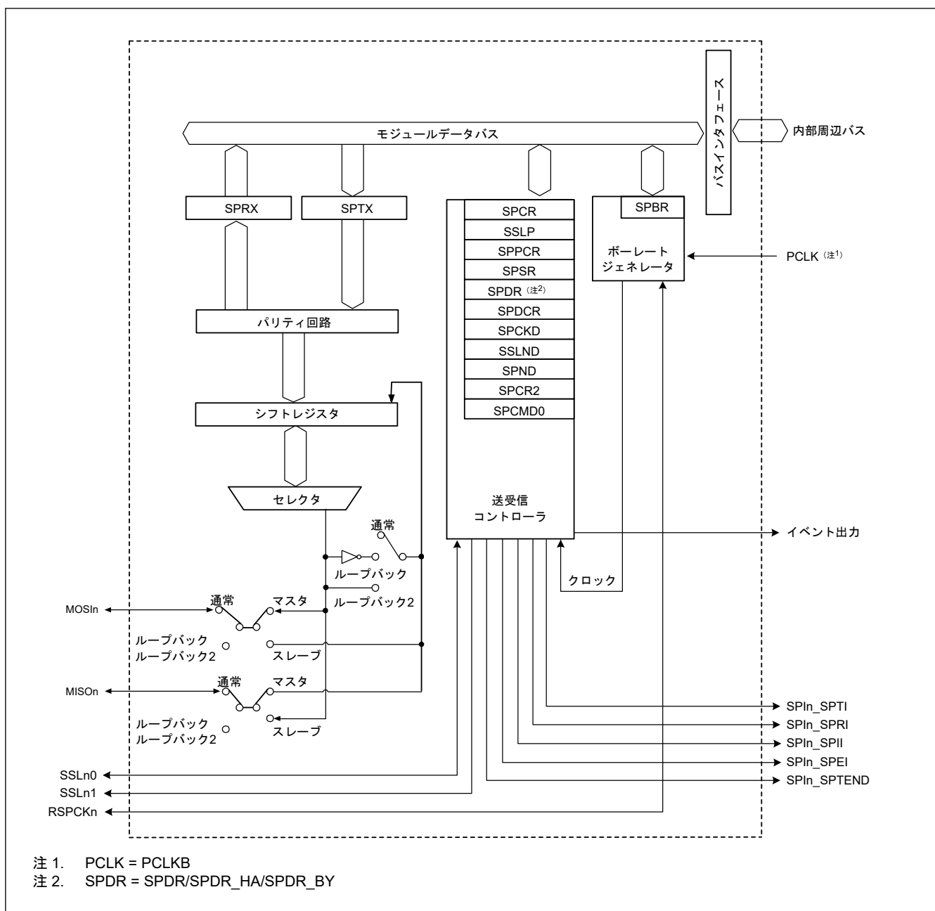
図 26.1 SPI のブロック図
