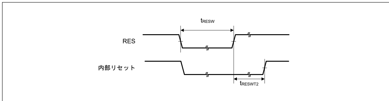
図 35.7 リセット入力タイミング (1)
