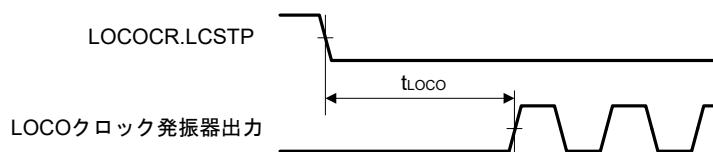
図 35.4 LOCO クロック発振開始タイミング
