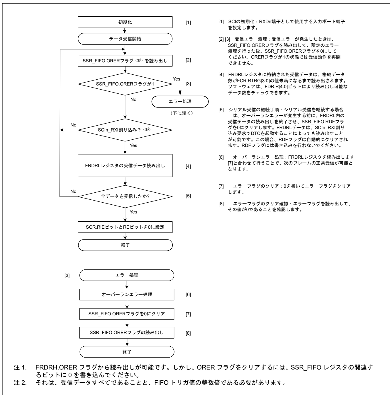
図 24.44 クロック同期式モードにおけるシリアル受信のフローチャート例 (FIFO 選択時)
