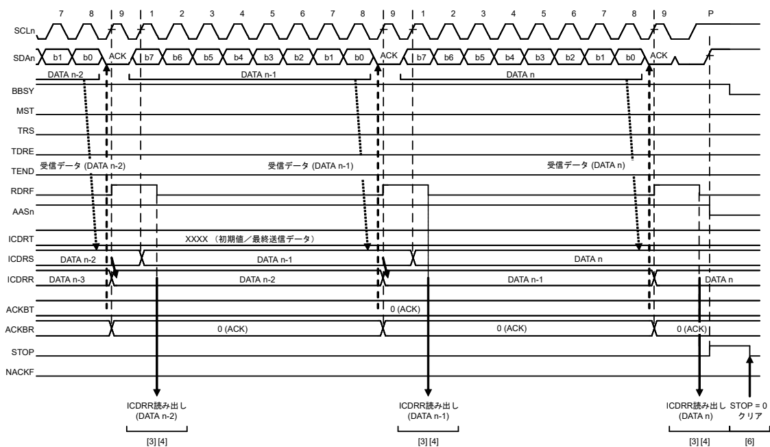
図 25.20 スレープ受信の動作タイミング (2) (RDRFS = 0 の場合)
