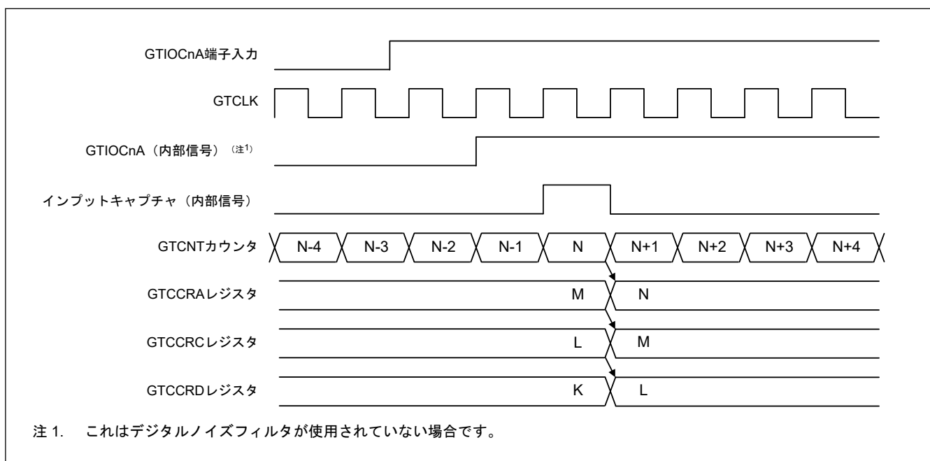
図 20.15 GTIOCN A 端子の入力の立ち上がりエッジに対応するインプットキャプチャ動作のタイミング例
