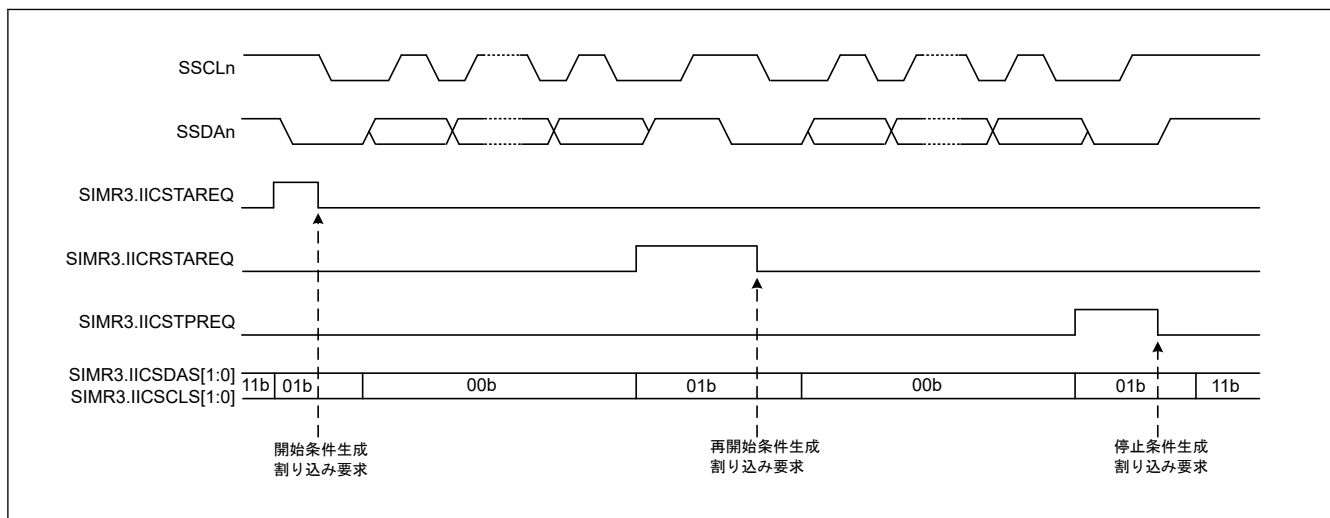
図 24.60 開始条件、再開始条件、停止条件生成の動作タイミング
