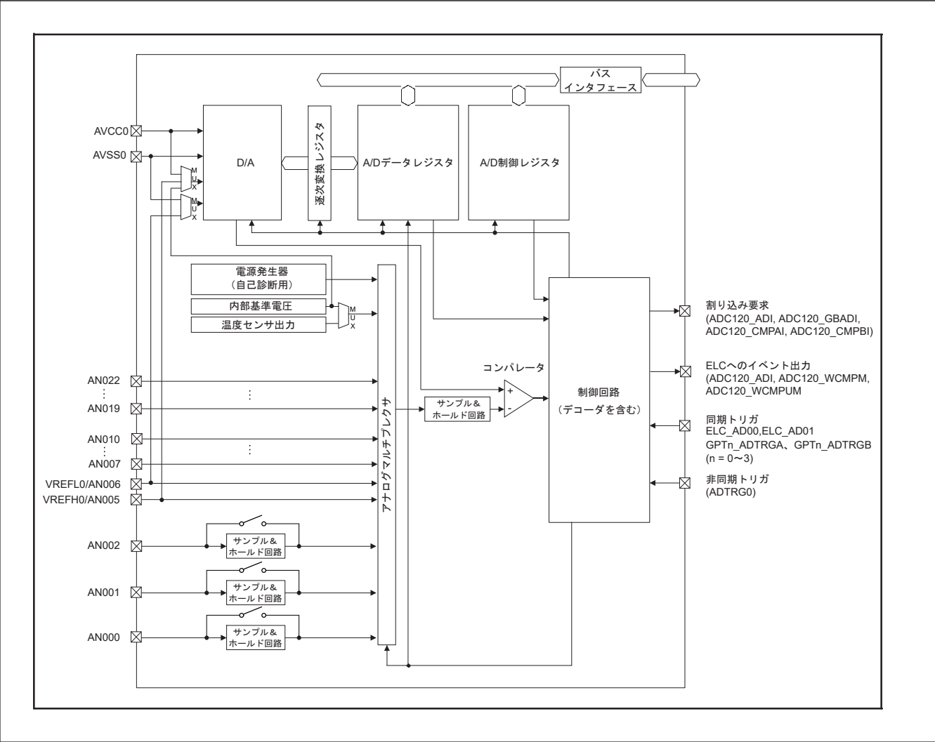
図 29.1 ADC12 のブロック図
