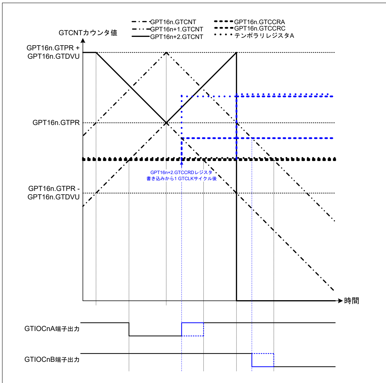
図 20.72 相補 PWM モード 4 のシングルバッファ動作例 (ダウンカウント山部分) (相補 PWM モード 4 のシングルバッファ動作、アップカウントの GTCCRA レジスタコンペアマッチ時: GTIOCN A 端子 = Low / GTIOCN B 端子 = High、ダウンカウントの GTCCRA レジスタコンペアマッチ時: GTIOCN A 端子 = High / GTIOCN B 端子 = Low、アップカウントのコンペアマッチ後ダウンカウントのコンペアマッチ前に GPT16n.GTCNT 値以上の値が GTCCRD レジスタに書き込まれた場合) ( n = 0 )
