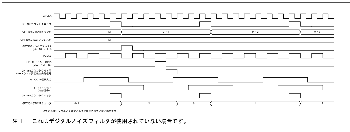
図 20.106 ELC_GPTA からのイベント入力に対応するカウンタクリアの動作タイミング例（ハードウェア要因によりトリガされるカウント中）
