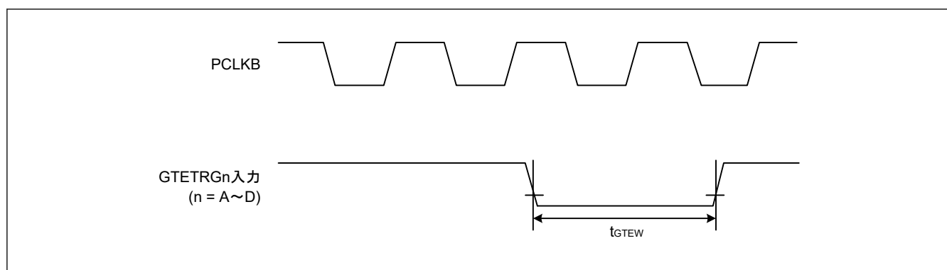
図 35.25 GPT 外部トリガ入力タイミング
