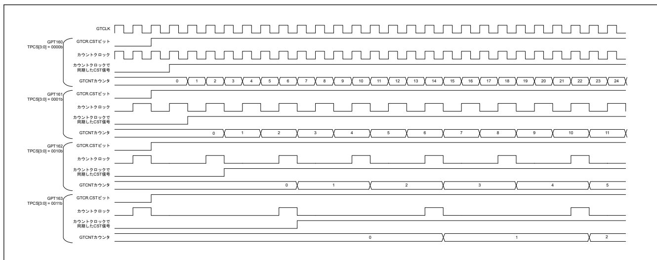
図 20.109 ソフトウェアによる同時スタートの動作例 (異なるカウント周期)
