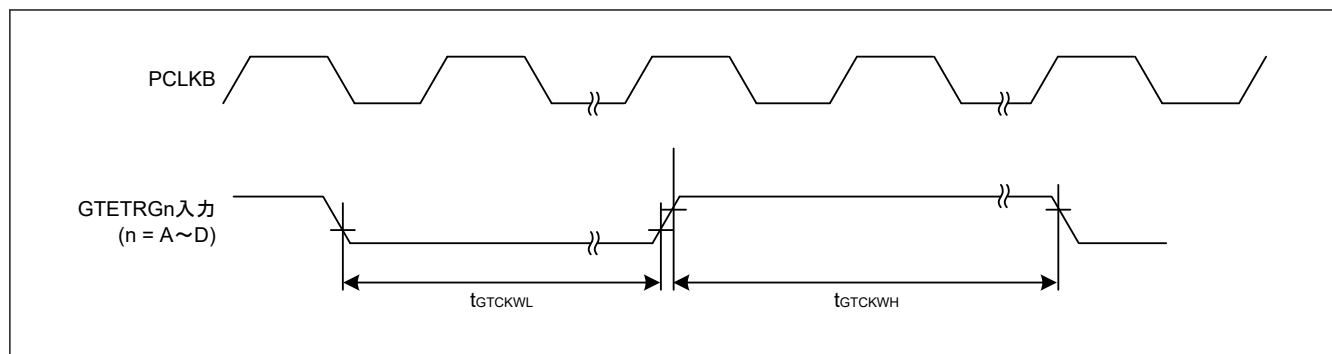
図 35.26 GPT クロック入力タイミング
