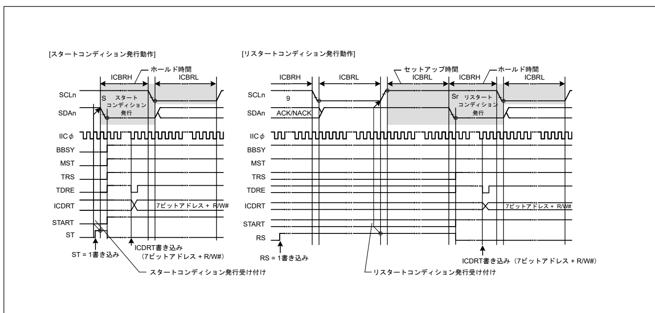
図 25.45 スタートコンディション/リスタートコンディション発行動作タイミング (ST、RS ビット)
