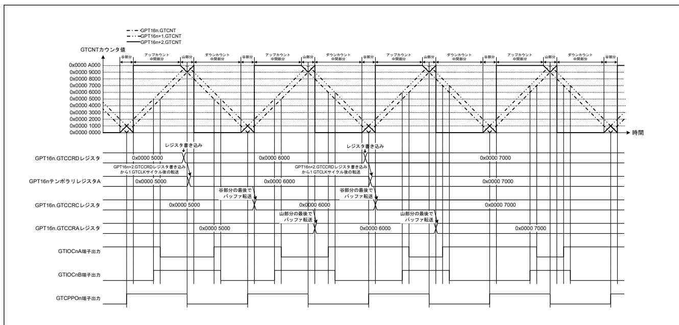
図 20.48 相補 PWM モード 1 動作例 (アップカウン트의 GTCCRA レジスタコンペアマッチ時 : GTIOCnA 端子 = Low/GTIOCnB 端子 = High、ダウンカウン트의 GTCCRA レジスタコンペアマッチ時 : GTIOCnA 端子 = High/GTIOCnB 端子 = Low、デッドタイム値 : 0x0000 1000、GTCCRD レジスタを山部分と谷部分で更新) (n = 0)
