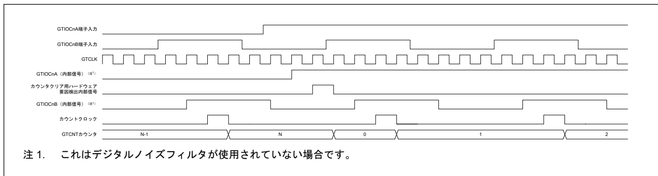
図 20.105 GTIOChA 端子入力の立ち上がりエッジに対応するカウンタクリアの動作タイミング例（ハードウェア要因によりトリガされるカウント中）
