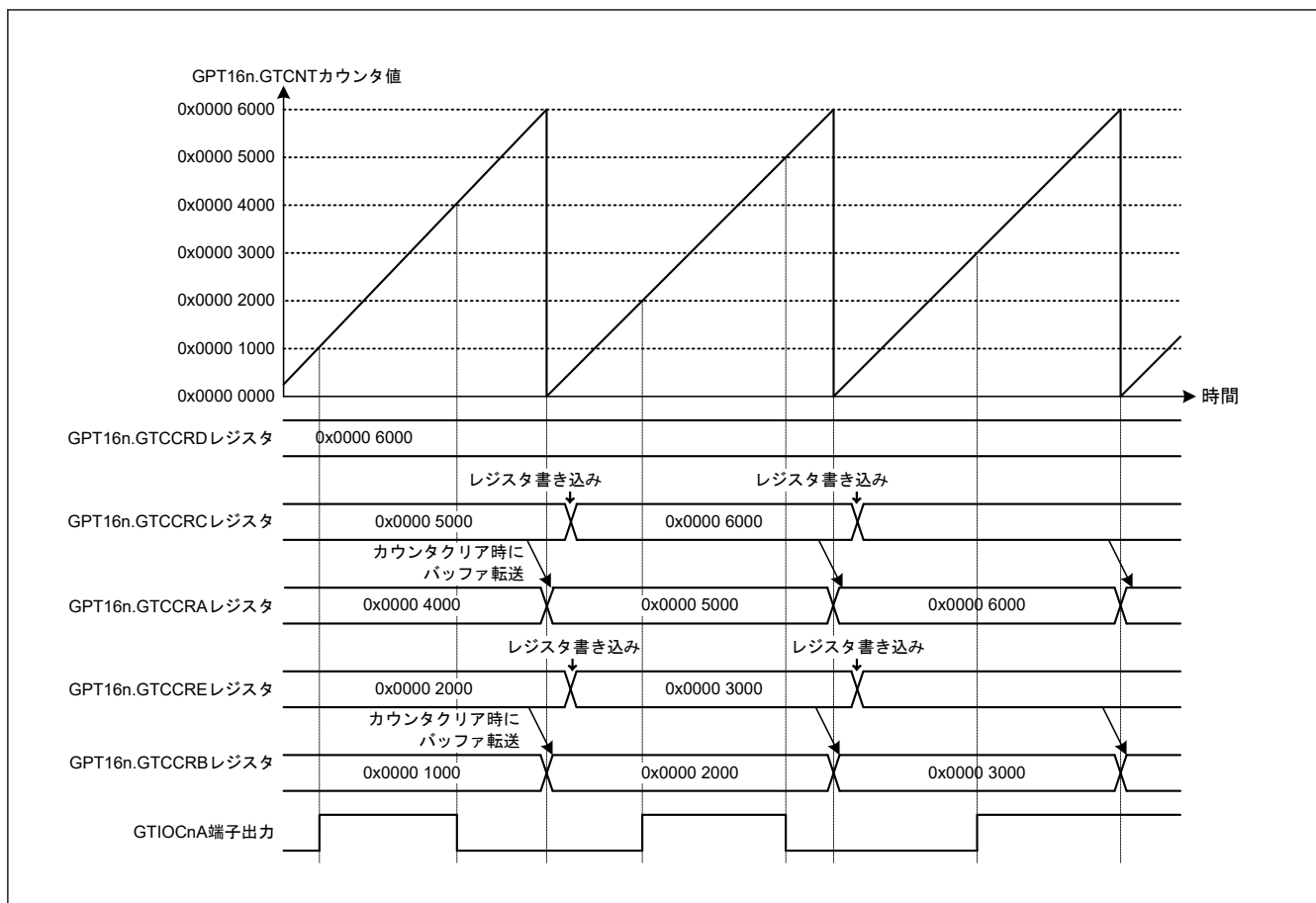
図 20.41 のこぎり波 PWM モード 2 の動作例 (GTCCRA レジスタコンペアマッチ時に Low 出力、GTCCRB レジスタコンペアマッチ時に High 出力、周期の終わりに Low 出力、シングルバッファ動作、GTCCRD レジスタコンペアマッチ時にクリア、GTIOR.OAEOCD ビット = 1) (n = 0~2)
