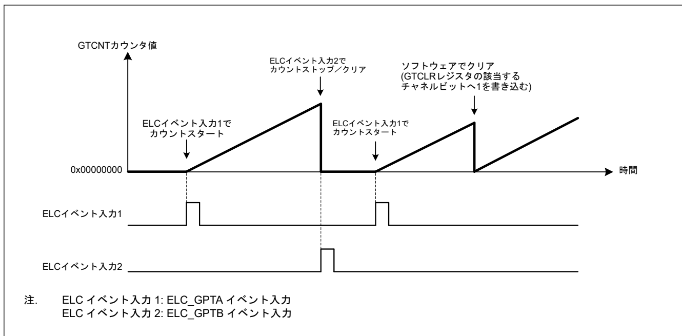
図 20.98 ハードウェア要因によるカウントクリア動作例 (のこぎり波アップカウント、ELC_GPTA 入力でスタート、ELC_GPTB 入力でストップ/クリアの場合)
