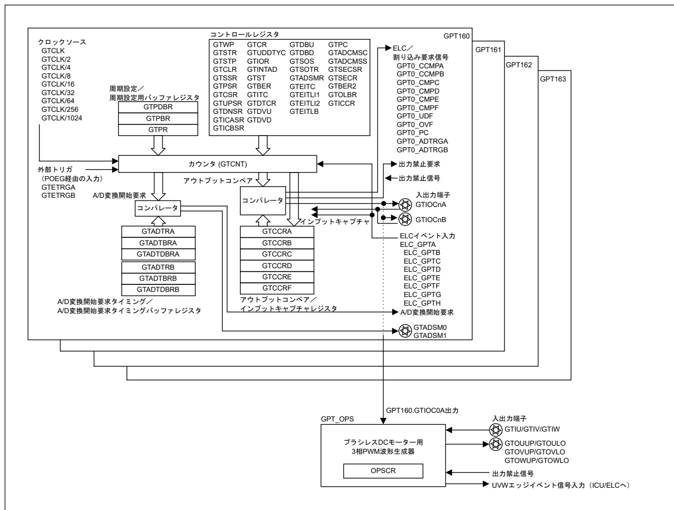
図 20.1 GPT のブロック図 (のこぎり波 PWM モード 1、のこぎり波ワンショットパルスモード、三角波 PWM モード 1、2、3)
