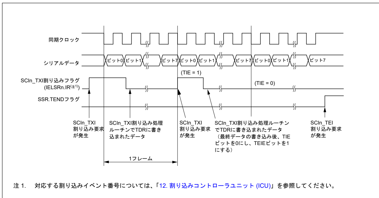
図 24.38 クロック同期式モードにおけるシリアル送信の動作例（送信中～送信終了時）
