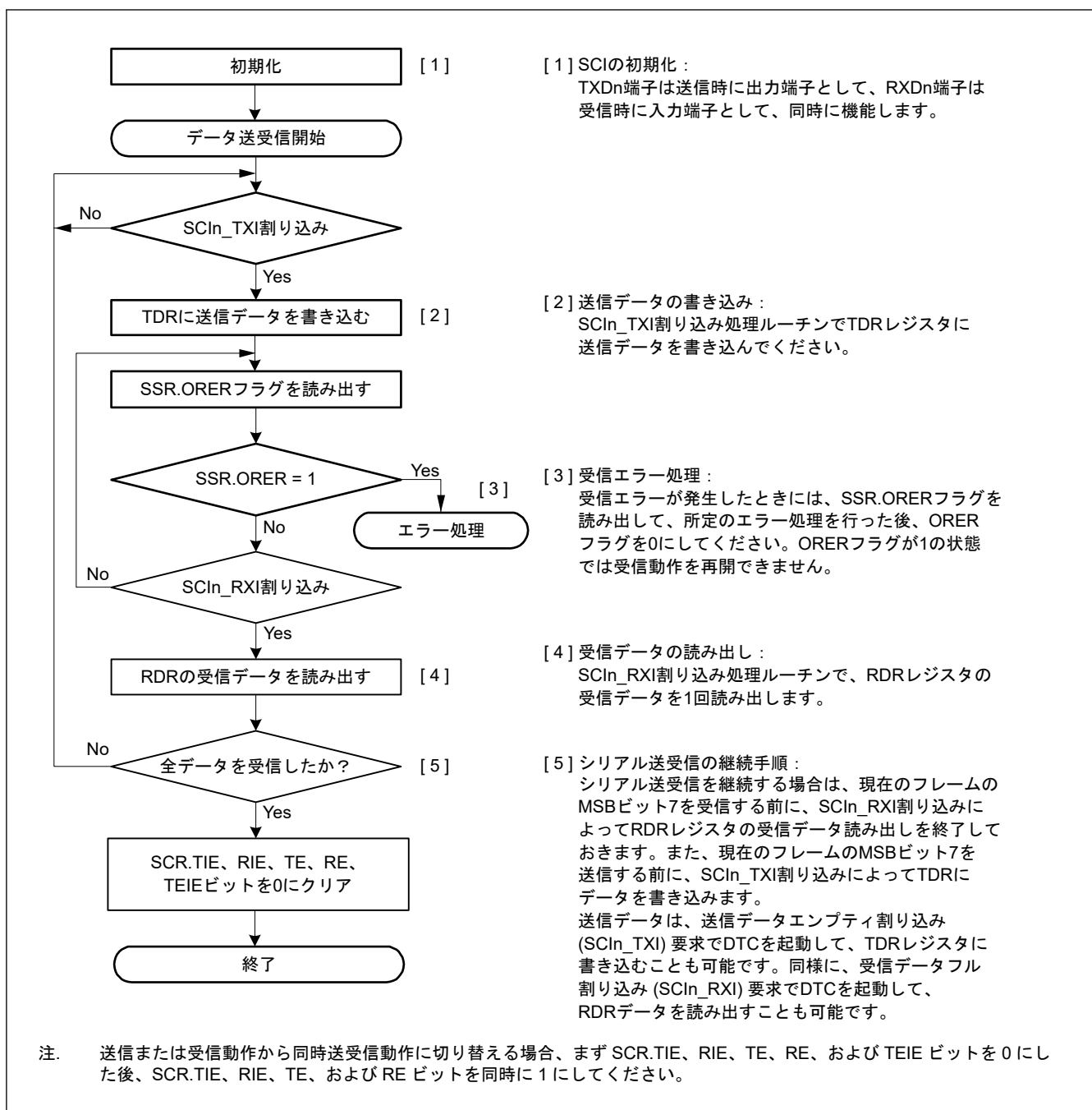
図 24.45 クロック同期式モードにおけるシリアル同時送受信動作のフローチャート例（非 FIFO 選択時）
