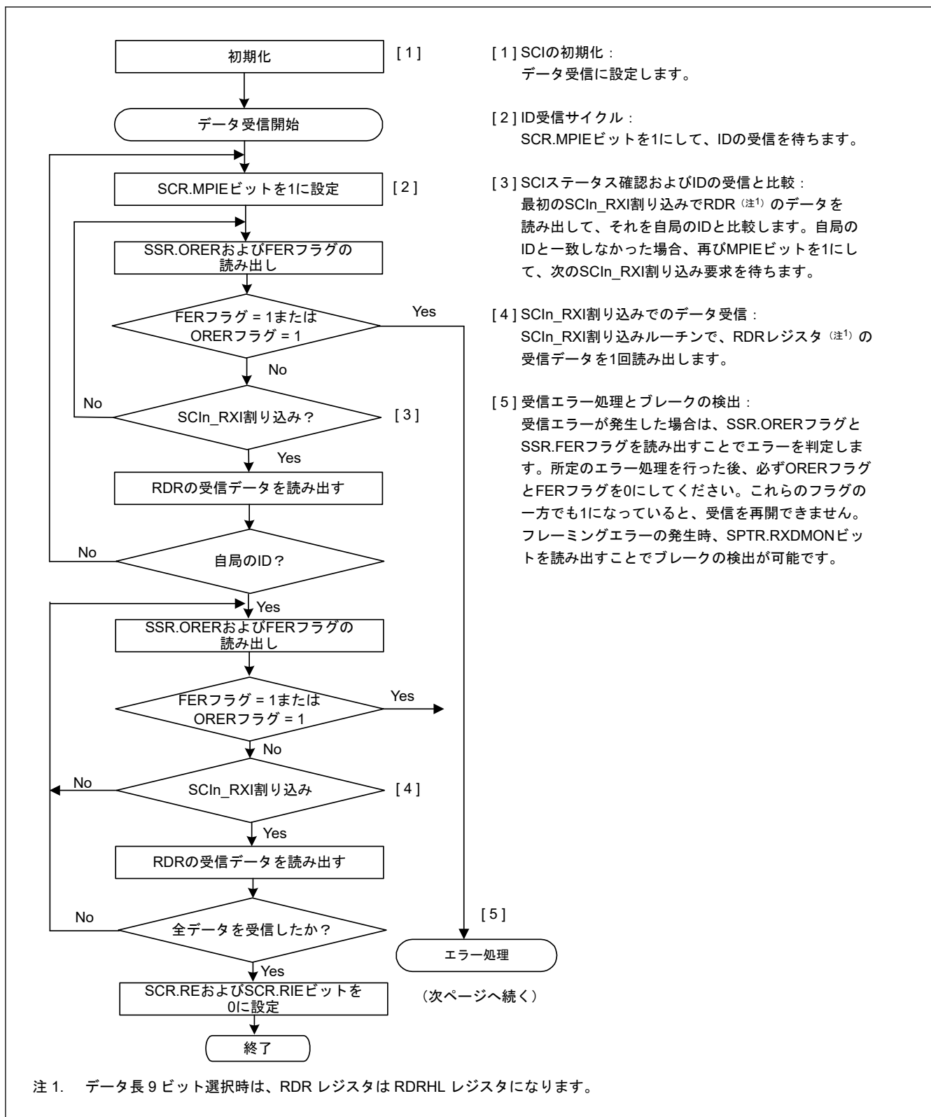
図 24.31 マルチプロセッサシリアル受信のフローチャート例（非 FIFO 選択時）(1)
