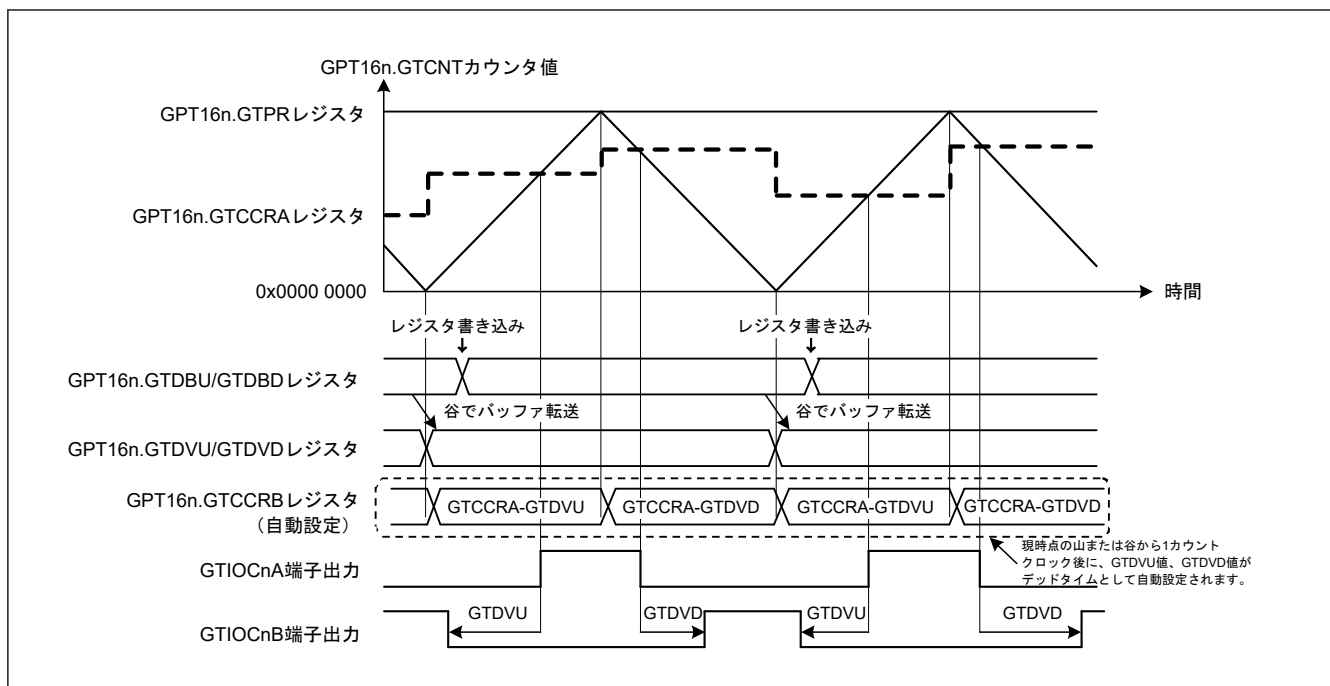
図 20.85 デッドタイム付きコンペアマッチ値の自動設定機能の動作例（三角波 PWM モード 2 または 3、GTDVU と GTDVD はバッファ動作に設定、GPT160～GPT162 でアクティブ High の場合）
