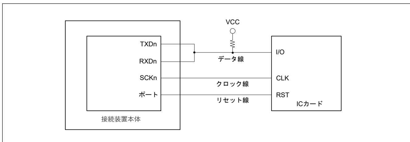
図 24.47 スマートカード (IC カード) との接続例
