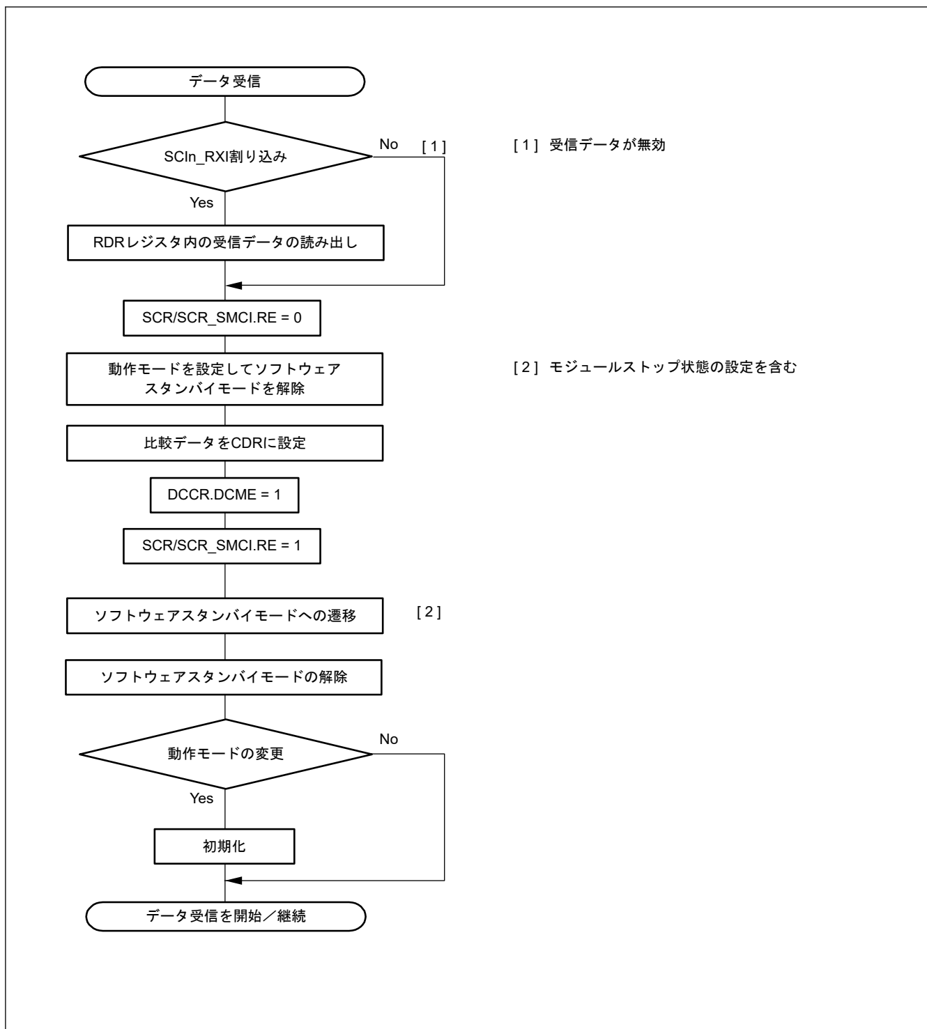
図 24.76 アドレス一致を用いて受信中にソフトウェアスタンバイモードへ遷移する場合のフローチャート例
