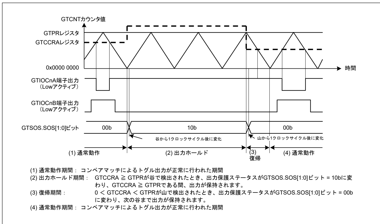
図 20.177 谷でのバッファ転送中に GTCCR \geq GTPR となったときの出力保護機能の動作例 (山でのバッファ転送中に 0 < GTCCR < GTPR に復帰、アクティブレベル : Low) ( n = 0 \sim 2 )
