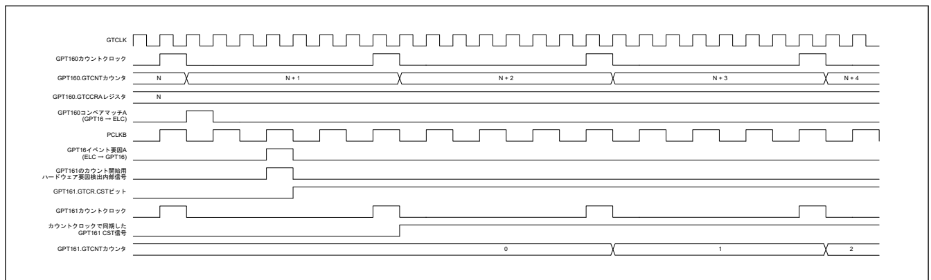
図 20.92 ELC_GPTA からのイベント入力に対応するカウントスタート動作のタイミング例
