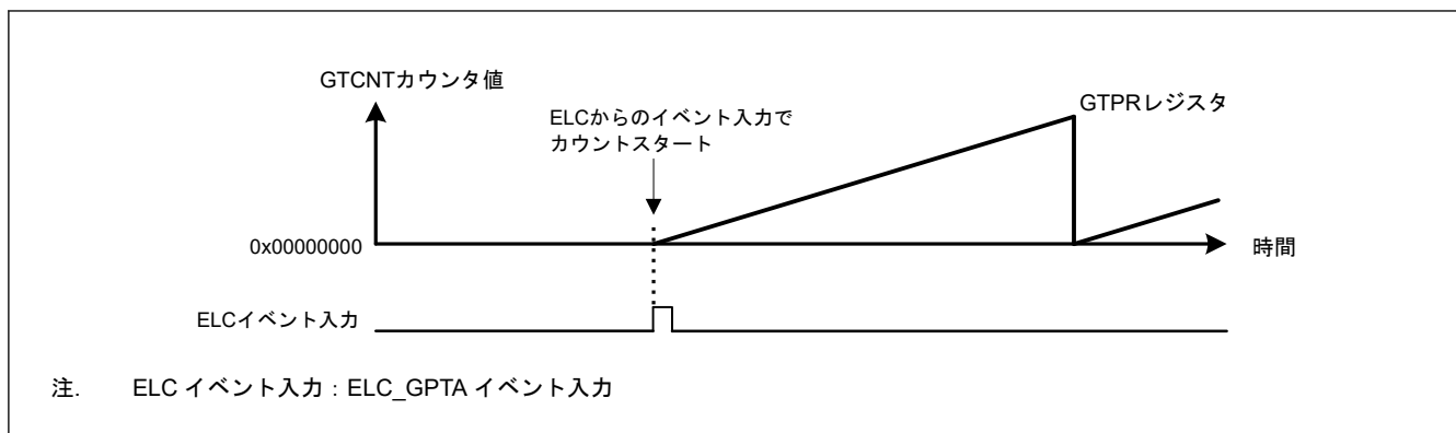
図 20.89 ハードウェア要因によるカウントスタート動作例 (ELC_GPTA イベントからの信号入力時のスタート)
