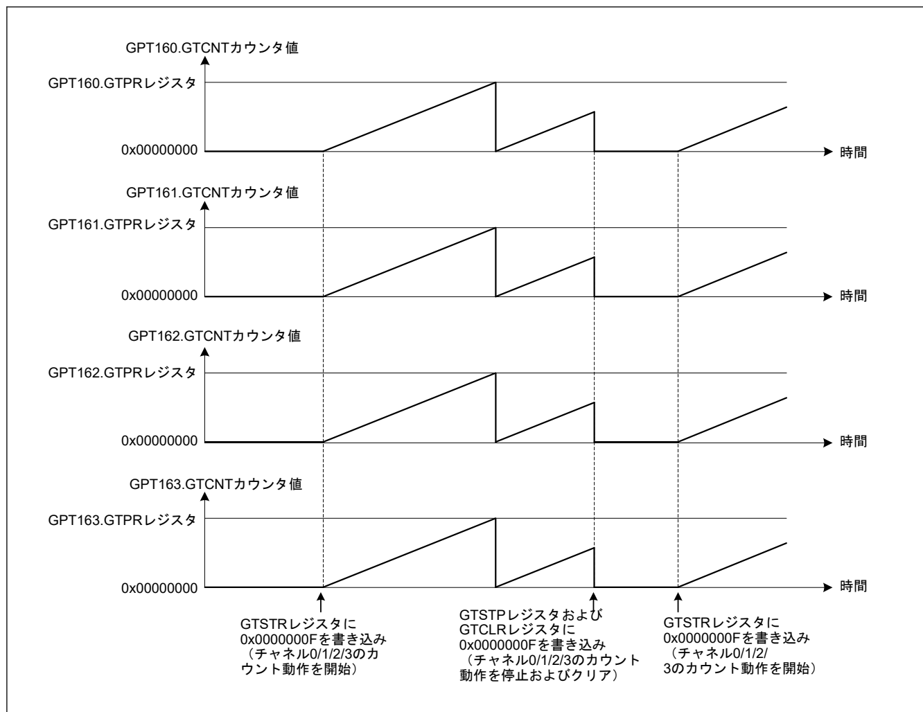
図 20.107 ソフトウェアによる同時スタート/ストップ/クリアの動作例 (カウント周期 (GTPR レジスタ値) が同一のとき)
