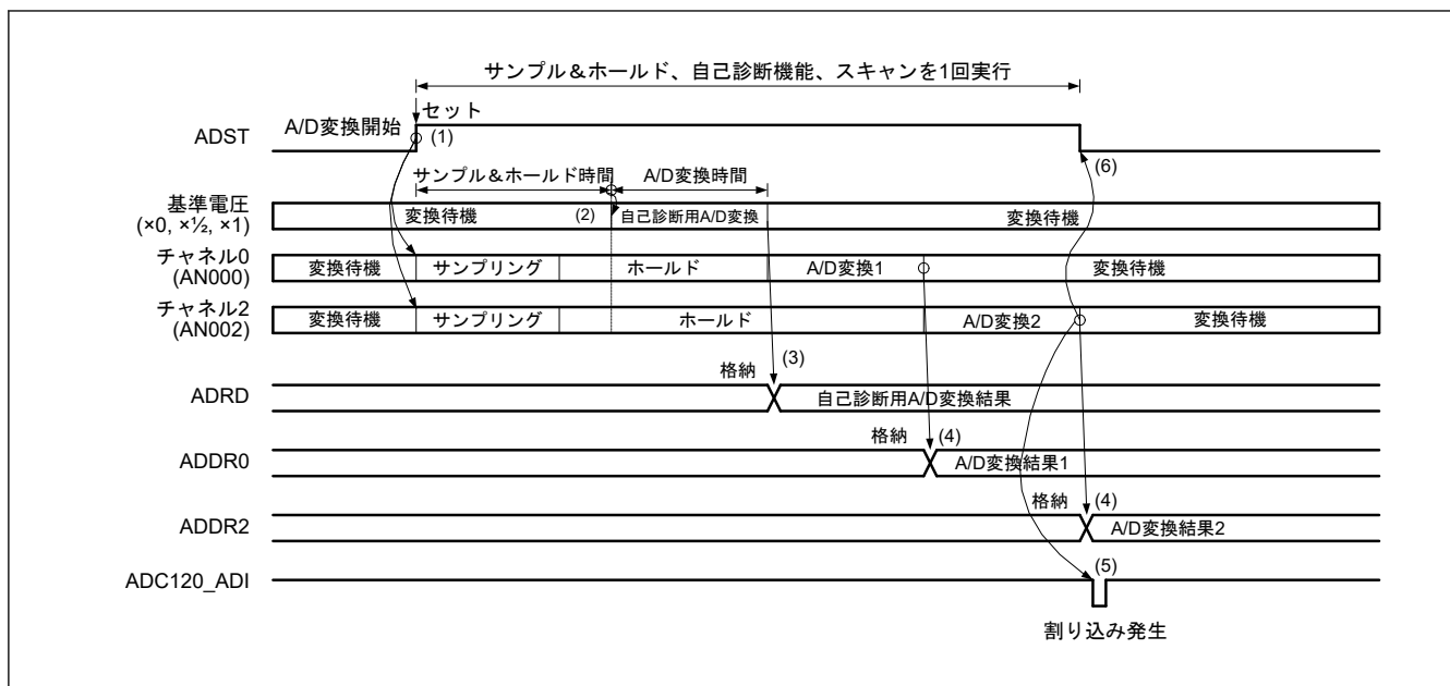
図 29.10 シングルスキャンモードの動作例 (チャンネル専用サンプル&ホールド回路使用、自己診断で AN000 および AN002 選択)
