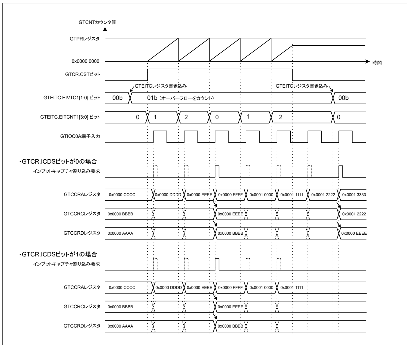
図 20.155 拡張割り込み間引き機能動作におけるインプットキャプチャの動作例（三角波でアップカウント、オーバーフローのカウン、拡張割り込み間引き 1 間引きカウン：2、EITCNT1 が 0 以外の期間での間引き、入力立ち上がりでインプットキャプチャ）
