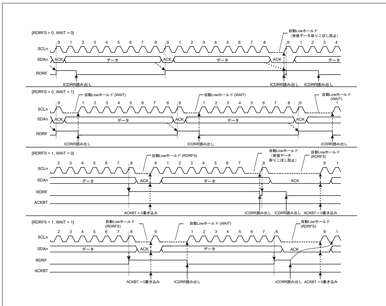
図 25.40 受信モード時の自動 Low ホールド動作 (RDRFS および WAIT ビットを使用)
