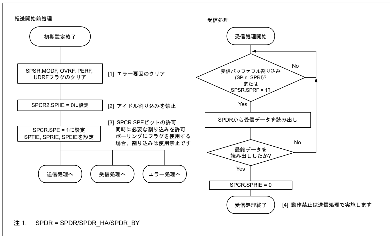
図 26.33 マスタモードでの受信フロー
