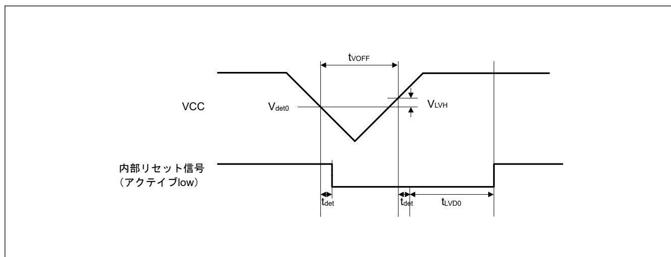
図 35.54 電圧検出回路タイミング ( V_{det0} )
