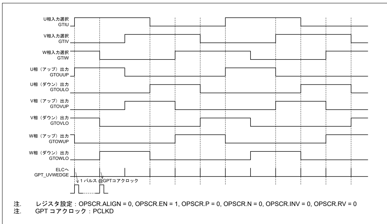
図 20.136 6 相レベル出力動作例
