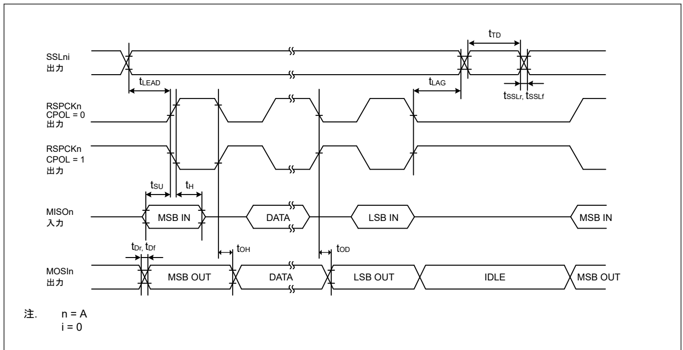
図 35.40 SPI タイミング (マスタ、CPHA = 0) (ビットレート : PCLKB を 2 分周以外に設定)
