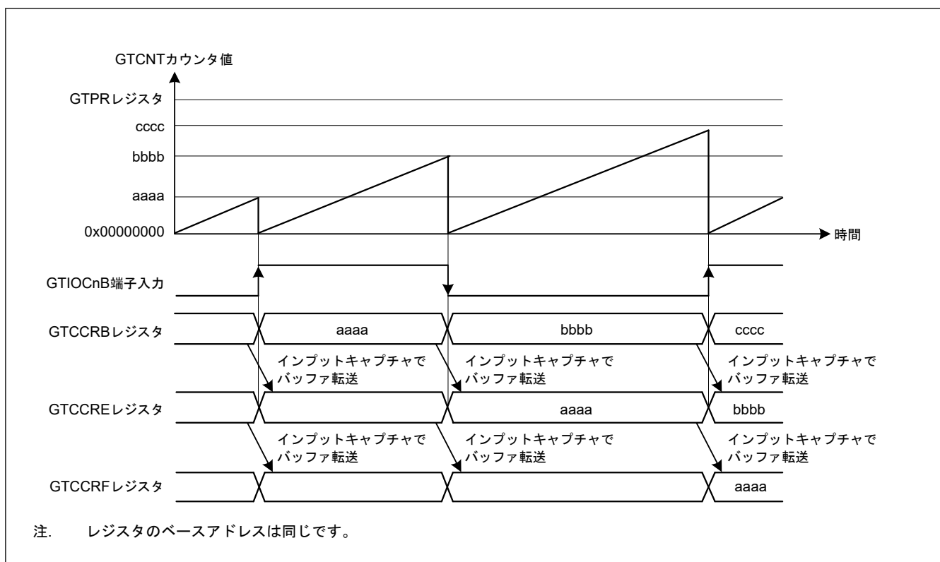
図 20.29 GTCCR A および GTCCR B レジスタのダブルバッファ動作例 (GTIOcNB 端子入力の両エッジでインプットキャプチャ、のこぎり波でアップカウント、GTIOcNB 端子入力の両エッジで GTCNT カウンタクリアの場合)
