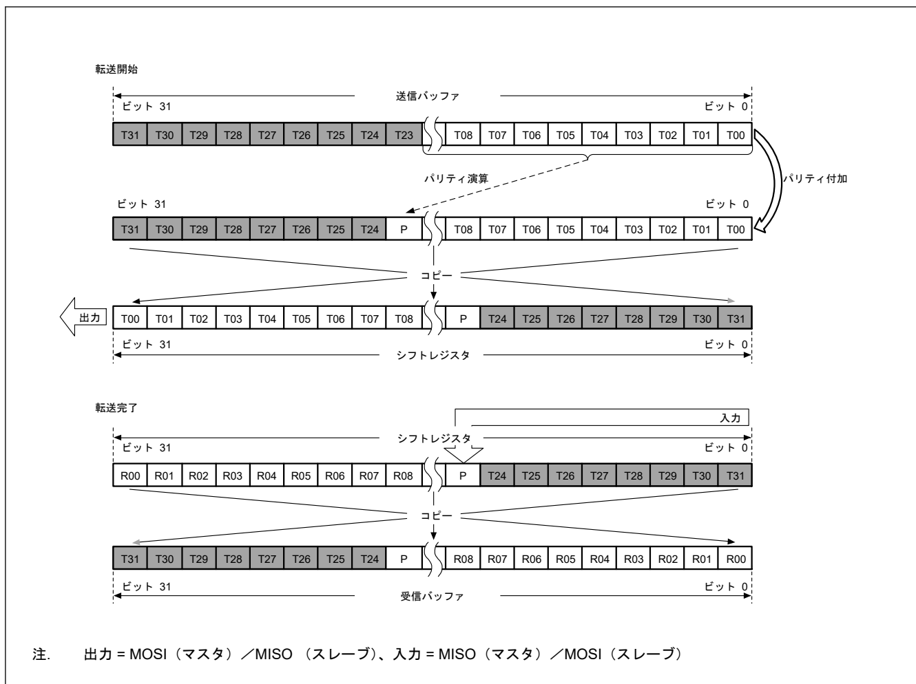
図 26.20 LSB ファースト転送 (24 ビットデータ/パリティ機能有効)
