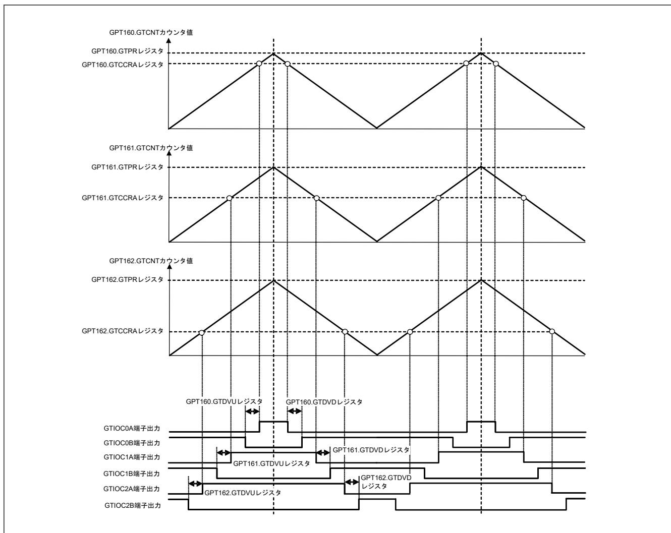
図 20.119 三角波 3 相相補 PWM 出力例（デッドタイム自動設定）
