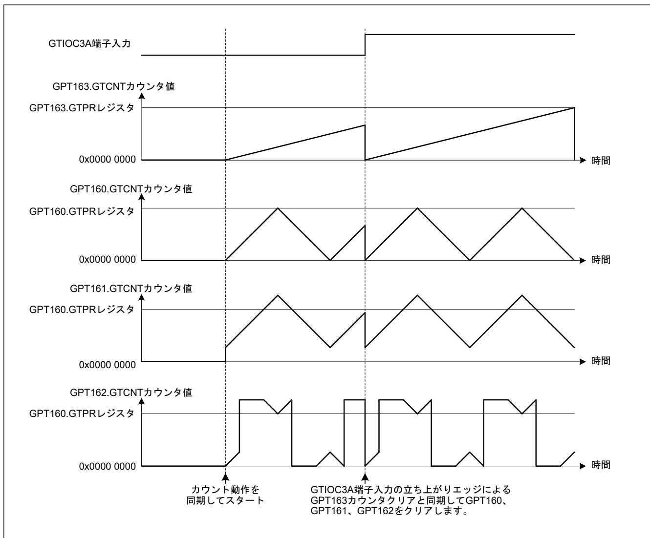
図 20.113 チャンネル間連携による同期クリアの動作例 (GTIOCnA/GTIOCnB 端子によるクリア) (GPT163 はのこぎり波で、カウンタは GTIOC3A の立ち上がりエッジによってクリアされます。GPT160、1、2 は相補 PWM モードです。GPT160、1、2、3 は同じ同期設定/クリアグループです)
