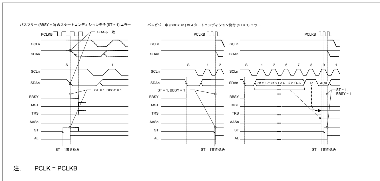
図 25.42 スタートコンディション発行時のアービトレーションロスト (MALE = 1 の場合)
