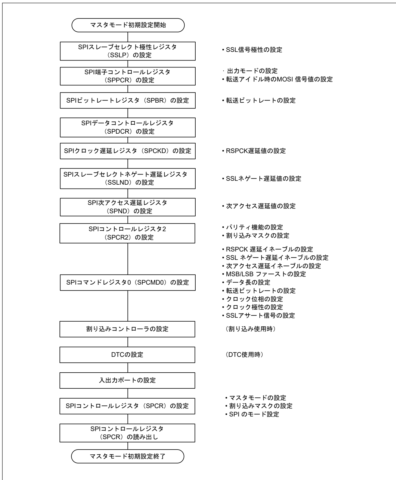
図 26.31 マスタモード時の SPI 動作の初期化フロー例
