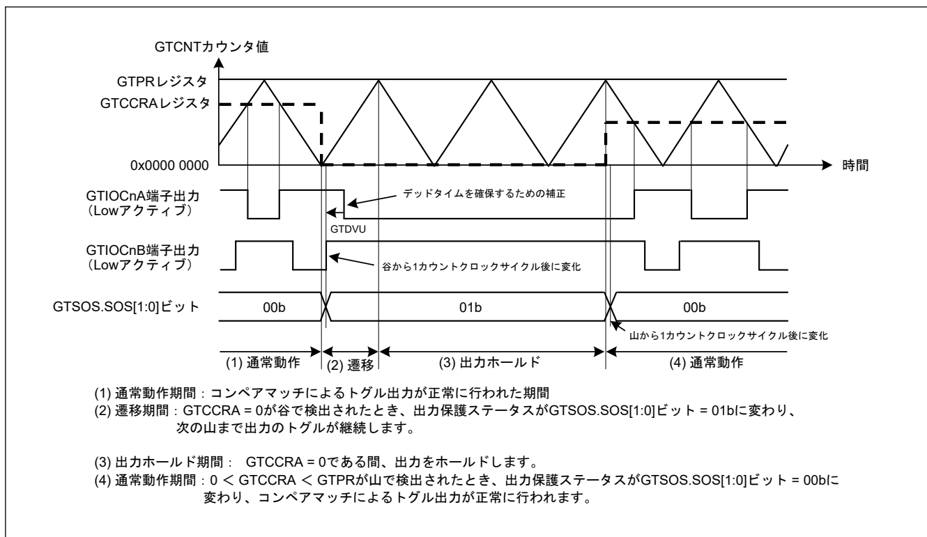
図 20.173 谷でのバッファ転送中に GTCCRA が 0x0000 0000 になったときの出力保護機能の動作例 (山でのバッファ転送中に 0 < GTCCRA < GTPR に復帰、アクティブレベル : Low) ( n = 0 \sim 2 )
