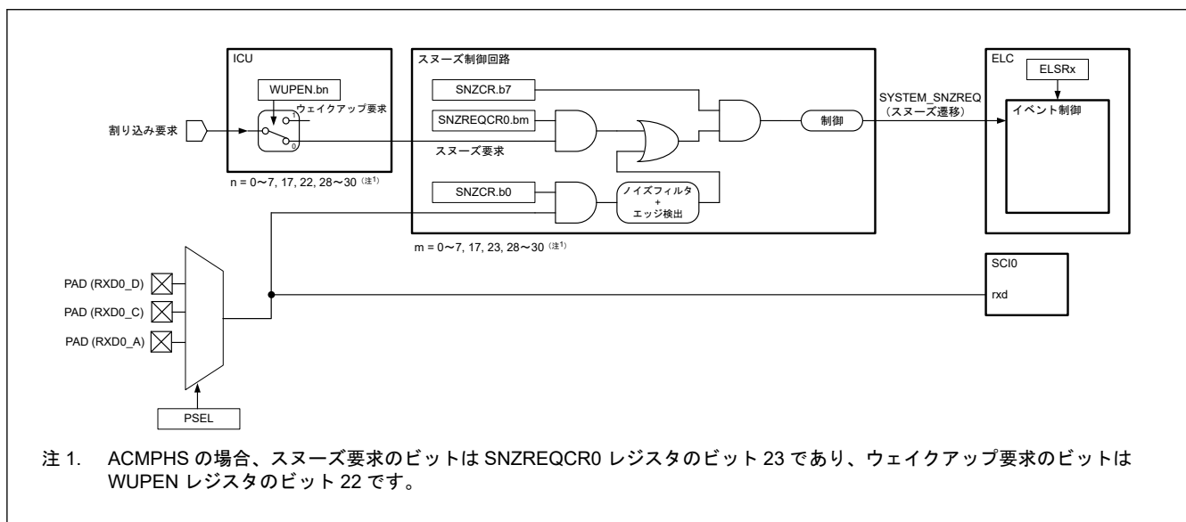
図 10.7 スヌーズモードへの遷移時構成
