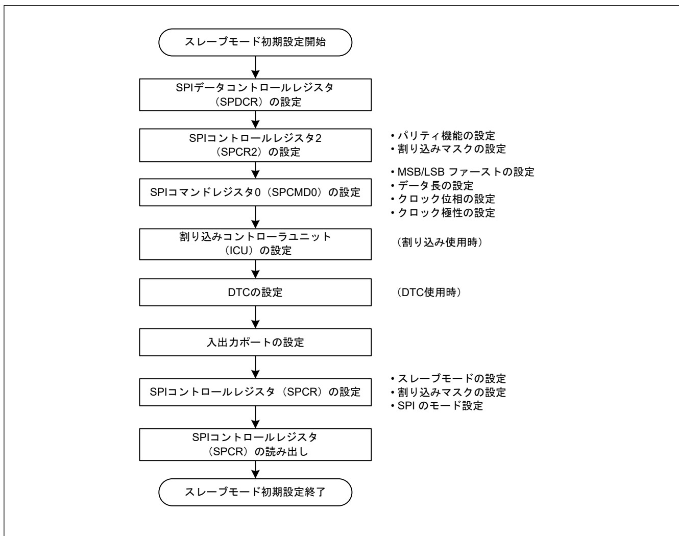
図 26.40 スレーブモード時のクロック同期式動作の初期化フロー例
