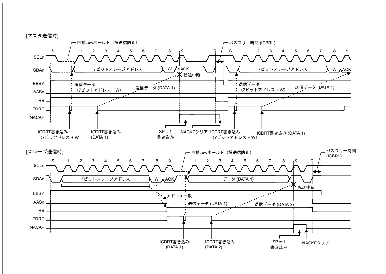
図 25.39 NACK 受信時のデータ転送中断動作 (NACK = 1 の場合)
