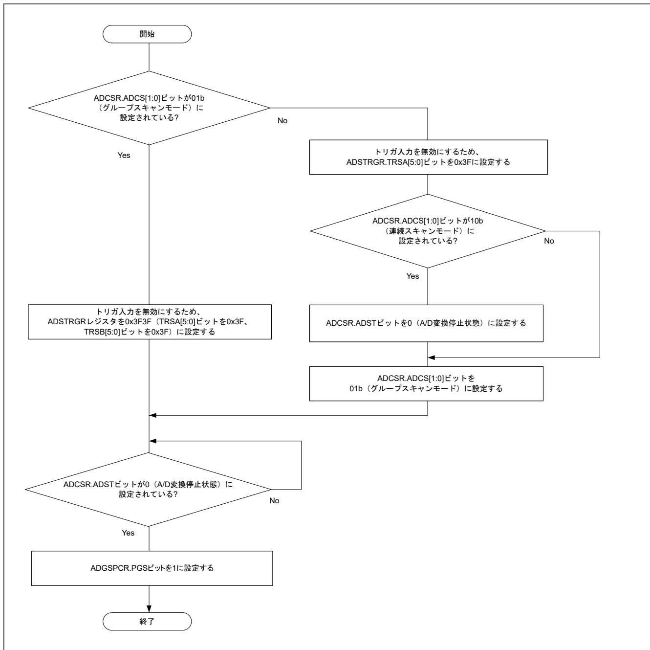
図 29.20 ADGSPCR.PGS ビット設定時のフローチャート
