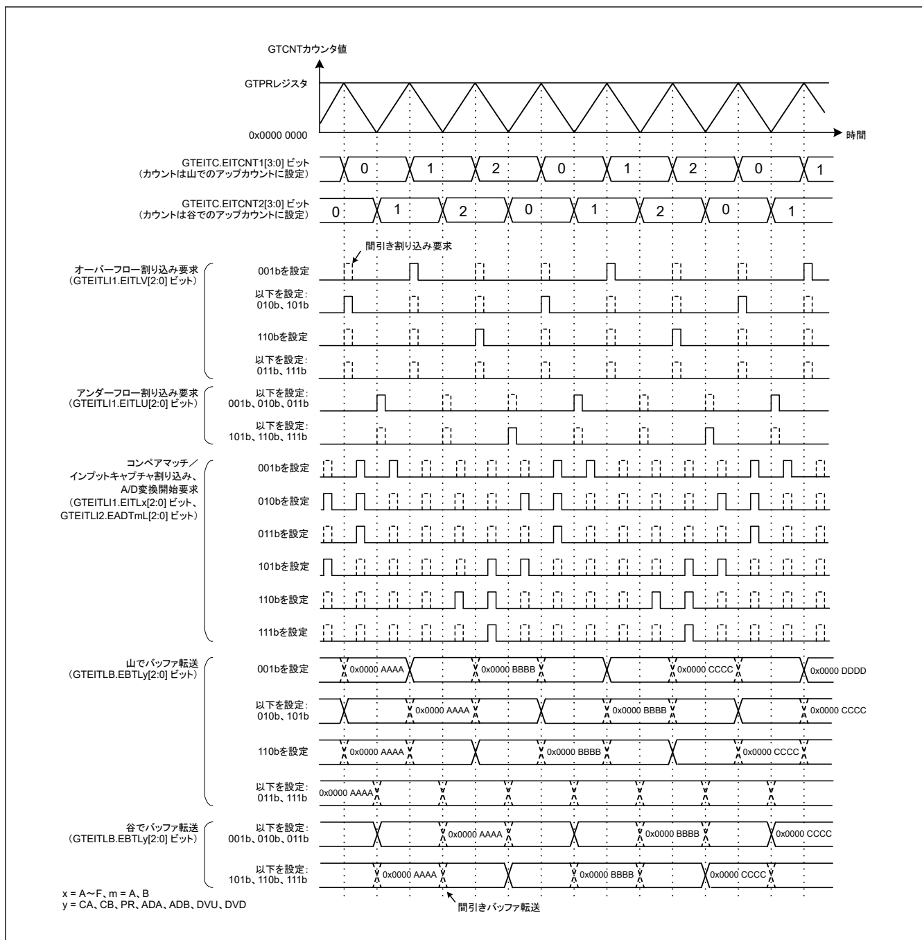
図 20.148 拡張割り込み間引き機能の例 (三角波、拡張割り込み間引き 1 による山でのカウント、間引きカウント : 2、拡張割り込み間引き 2 による谷でのカウント、間引きカウント : 2、拡張割り込み間引きカウンタ 2 の初期値 : 1)
