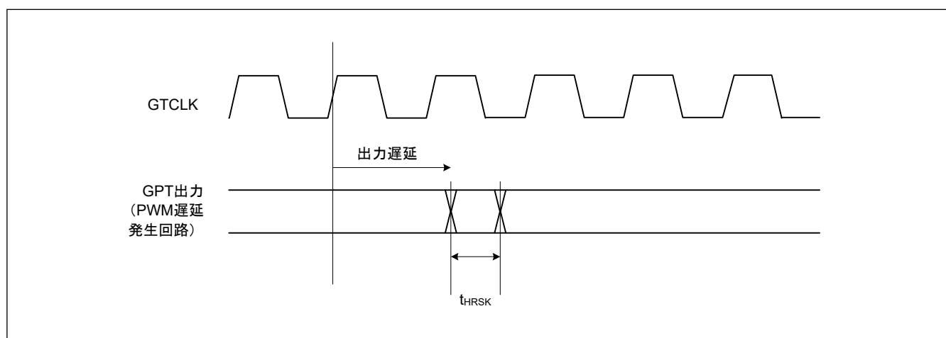
図 35.27 GPT (PDG) 出力遅延スキュー
