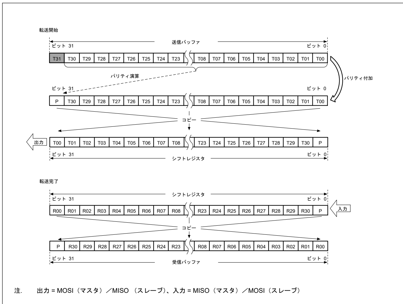
図 26.19 LSB ファースト転送 (32 ビットデータ/パリティ機能有効)
