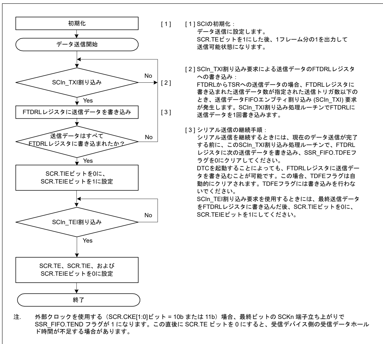
図 24.40 クロック同期式モードにおけるシリアル送信のフローチャート例 (FIFO 選択時)
