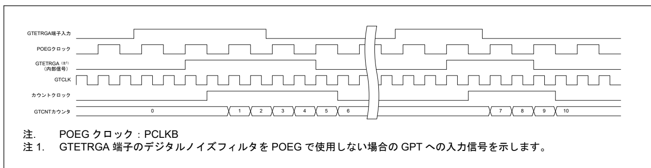
図 20.133 外部パルス幅測定機能の例 (アップカウント)
