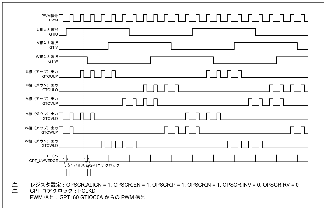
図 20.137 6 相 PWM 出力動作例 (チョップパ制御)
