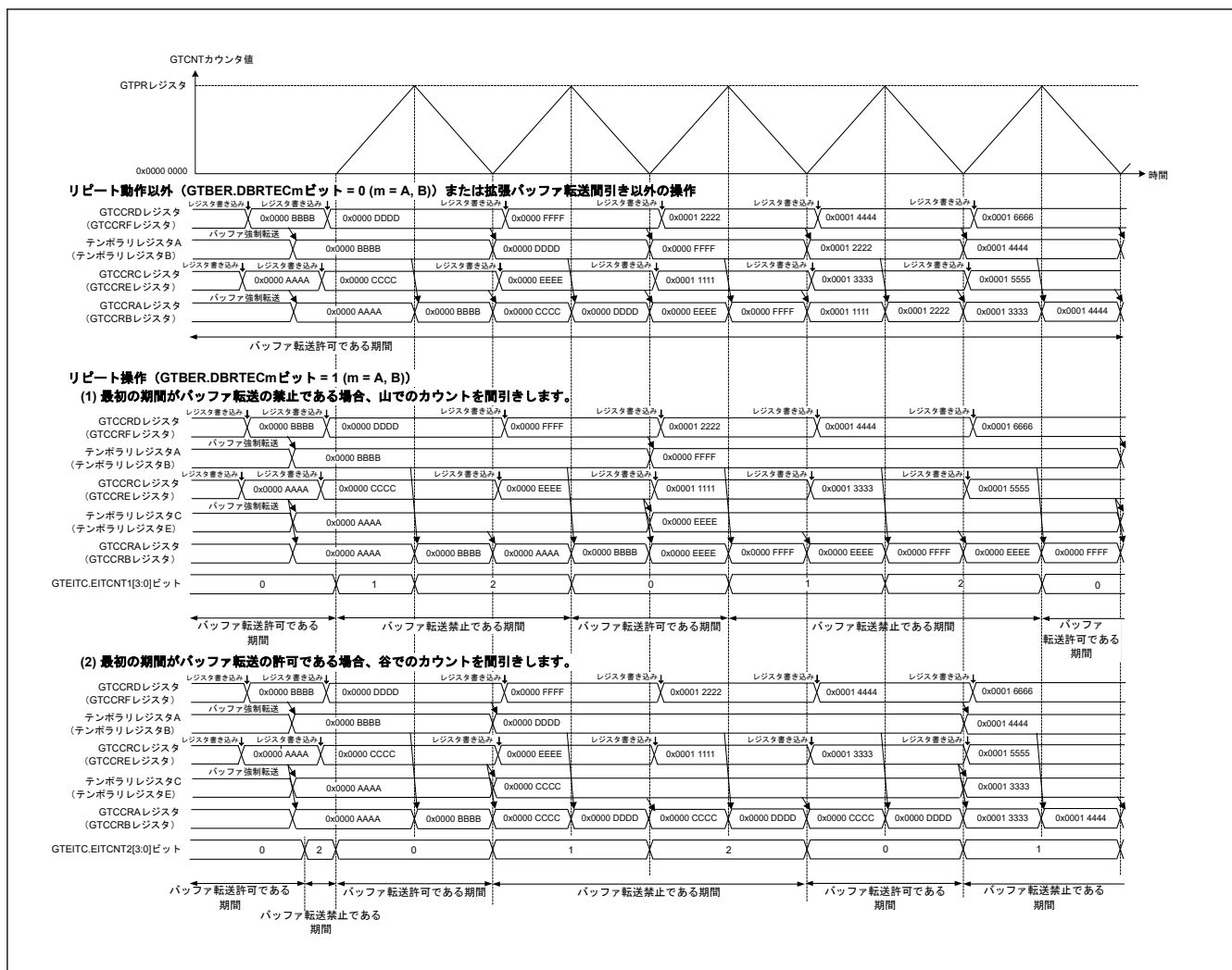
図 20.168 GTCCR バッファ転送が禁止されているときのリポートダブルバッファ動作例（三角波 PWM モード 3、拡張バッファ転送間引きを使用、GTBER.BD[0]は常に 0 の場合）
