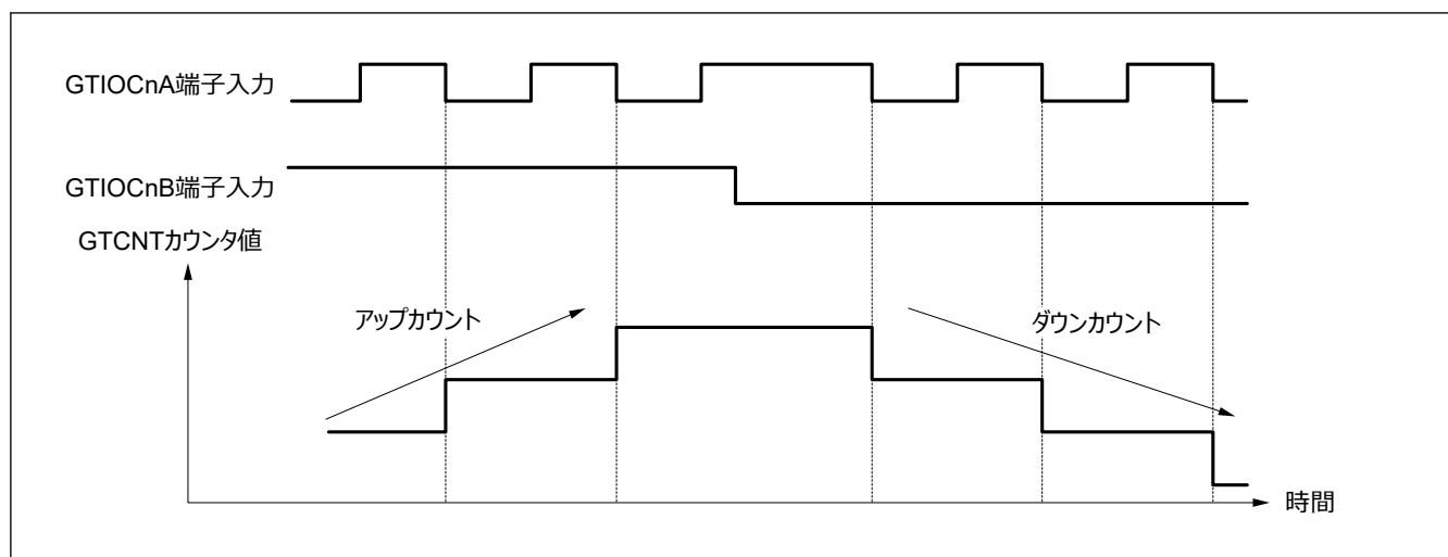
図 20.124 位相計数モード 2 の動作例 (A)
