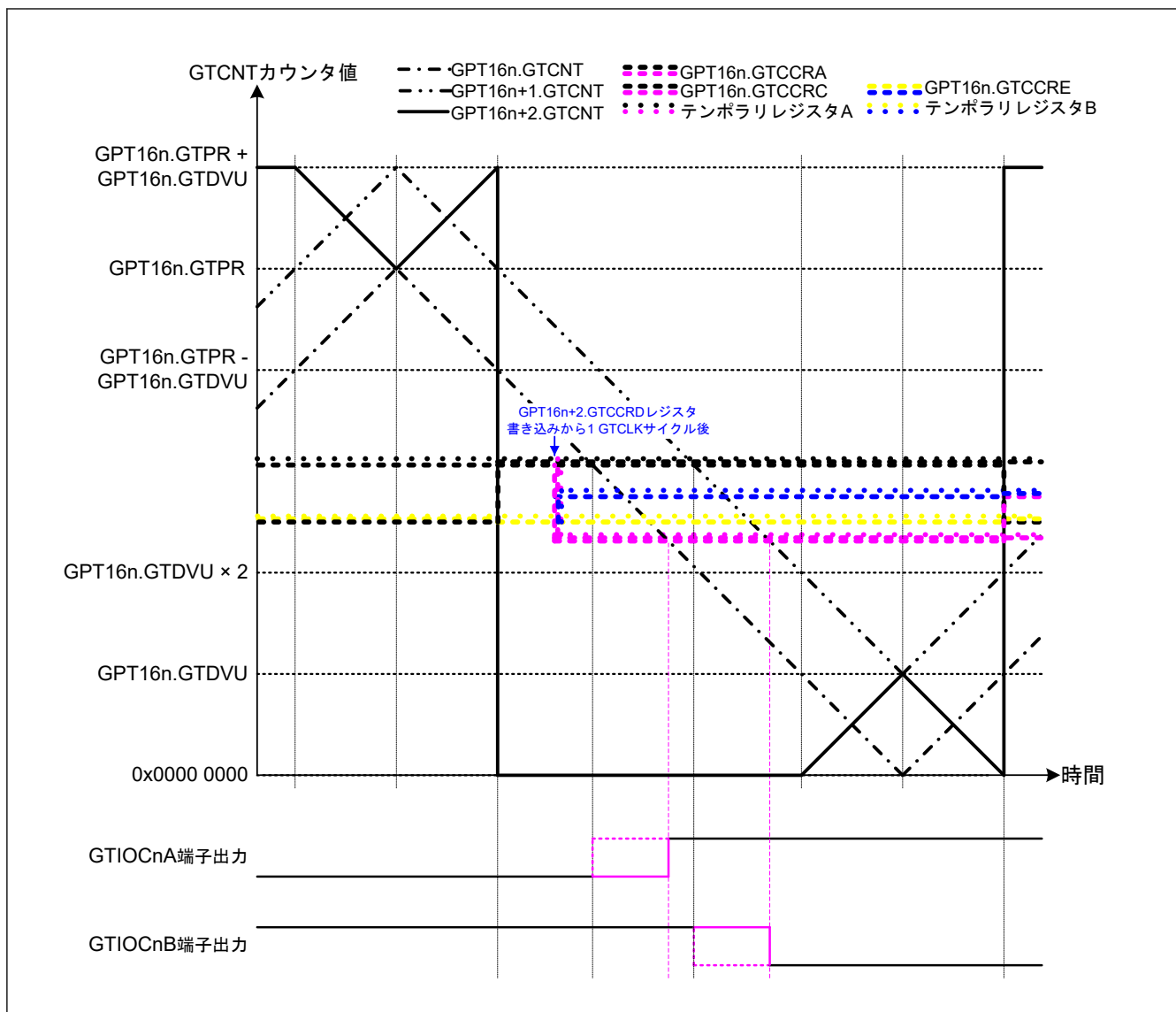
図 20.77 相補 PWM モード 4 のダブルバッファ動作の例 (ダウンカウント中間部分) (相補 PWM モード 4 のダブルバッファ動作、ダウンカウントの GTCCRA レジスタコンペアマッチ時: GTIOcNA 端子 = Low / GTIOcNB 端子 = High、ダウンカウントの GTCCRA レジスタコンペアマッチ時: GTIOcNA 端子 = High / GTIOcNB 端子 = Low、ダウンカウントのコンペアマッチ前に GPT16n.GTCNT 値よりも小さい値が GTCCRD レジスタに書き込まれた場合) (n = 0)
