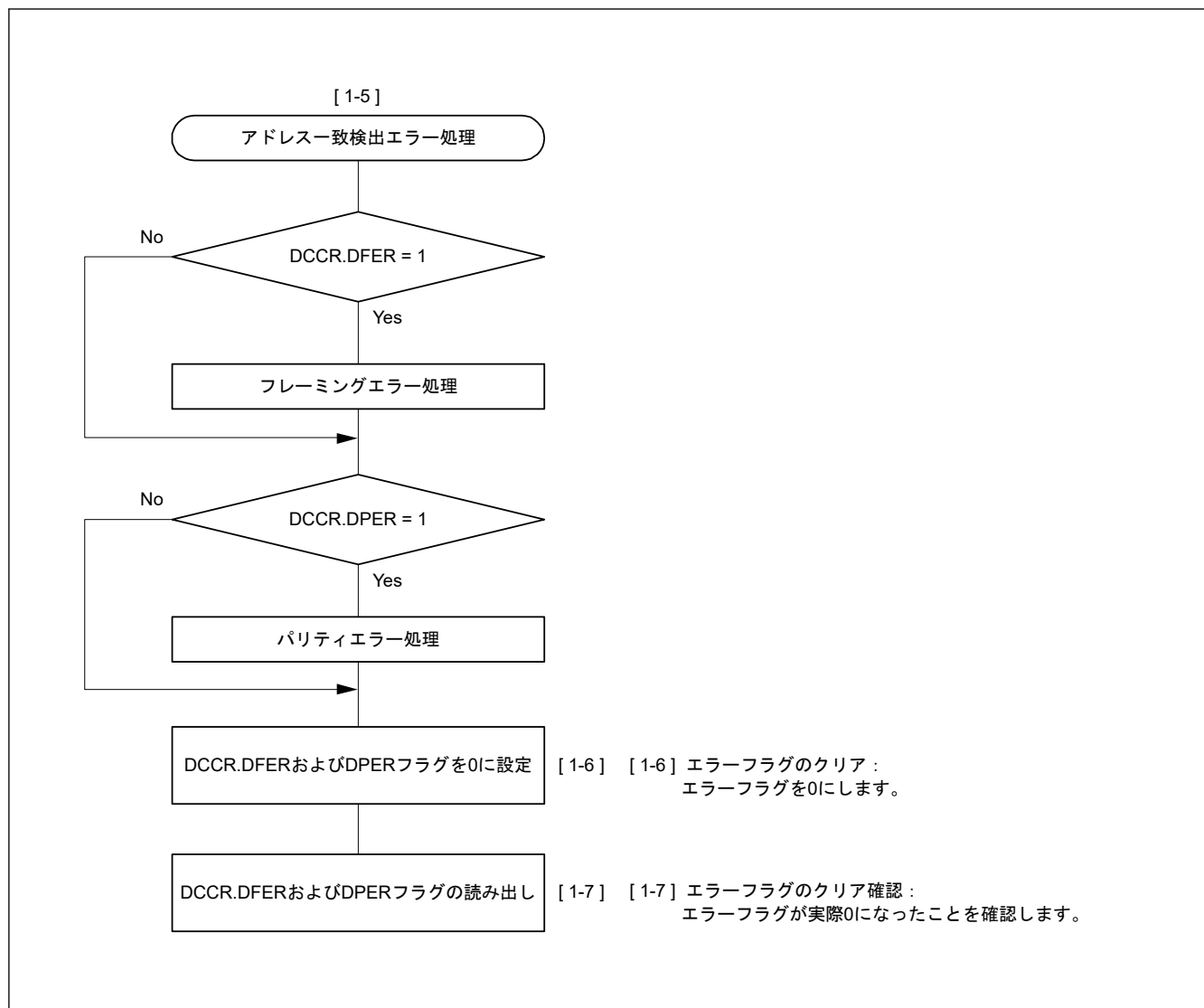
図 24.24 調歩同期式モードにおけるシリアル受信のフローチャート例 (FIFO 選択、アドレス一致検出有効時) (2)
