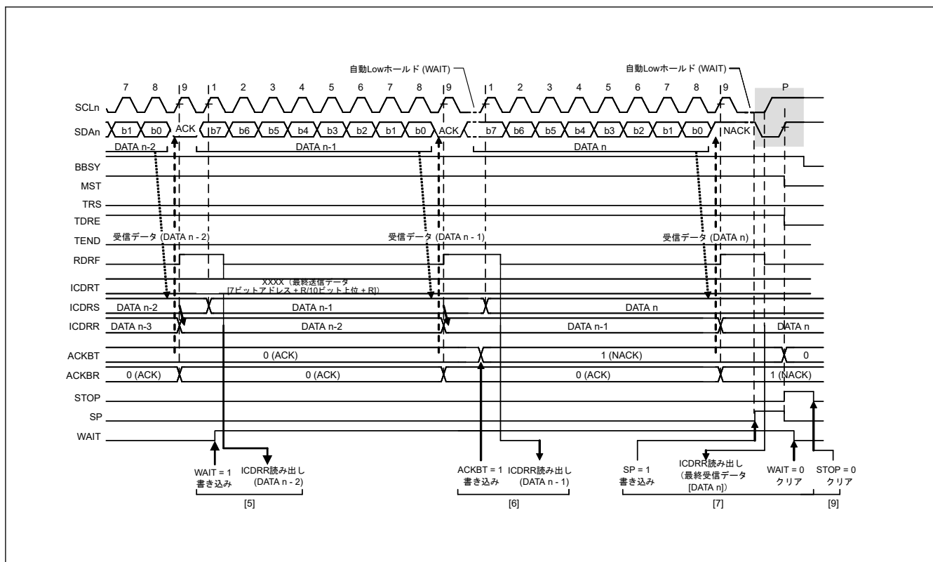
図 25.14 マスタ受信の動作タイミング (3) (RDRFS = 0 の場合)
