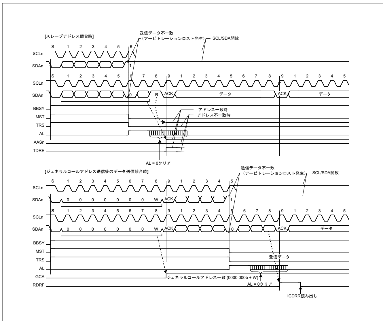
図 25.41 マスタアービトレーションロスト検出動作例 (MALE = 1 の場合)
