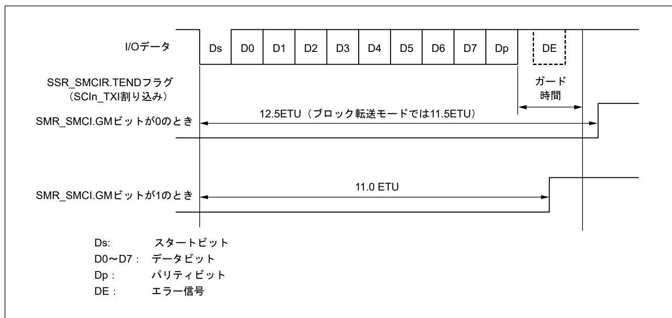
図 24.53 送信中の SSR.TEND フラグの発生タイミング
