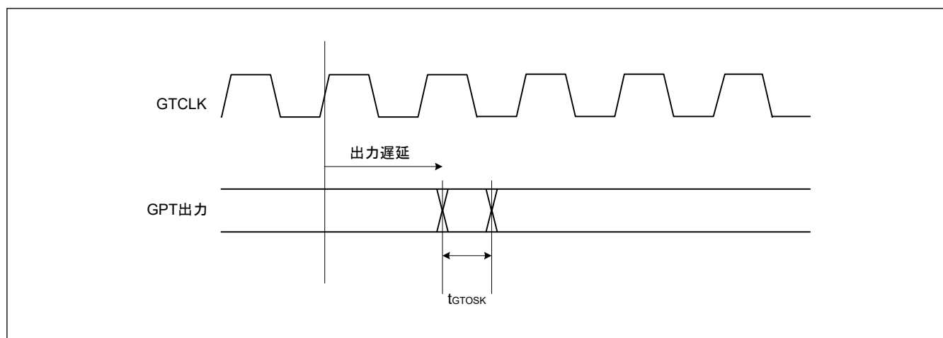
図 35.24 OPS の GPT 出力遅延スキュー
