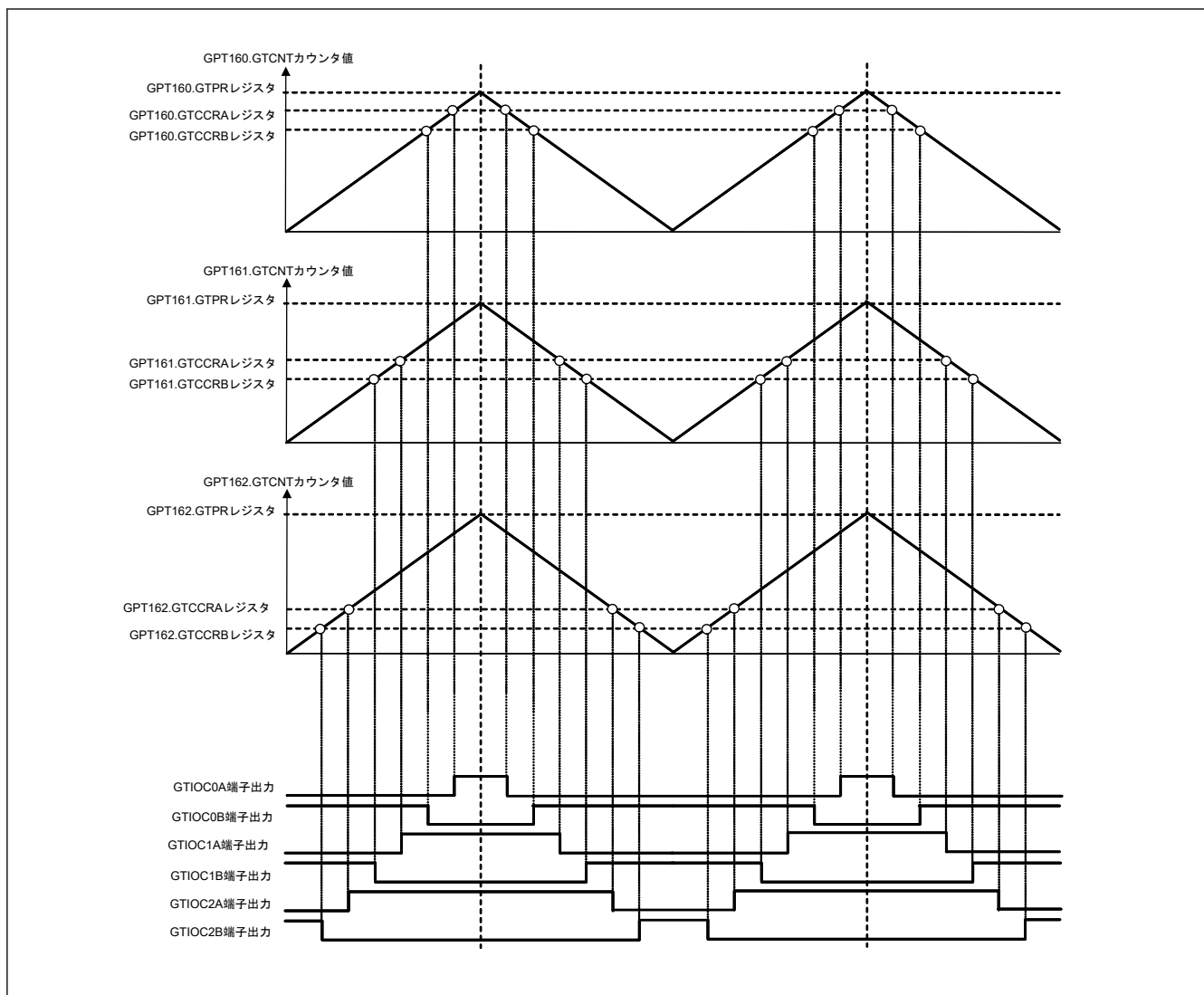
図 20.118 三角波 3 相相補 PWM 出力例
