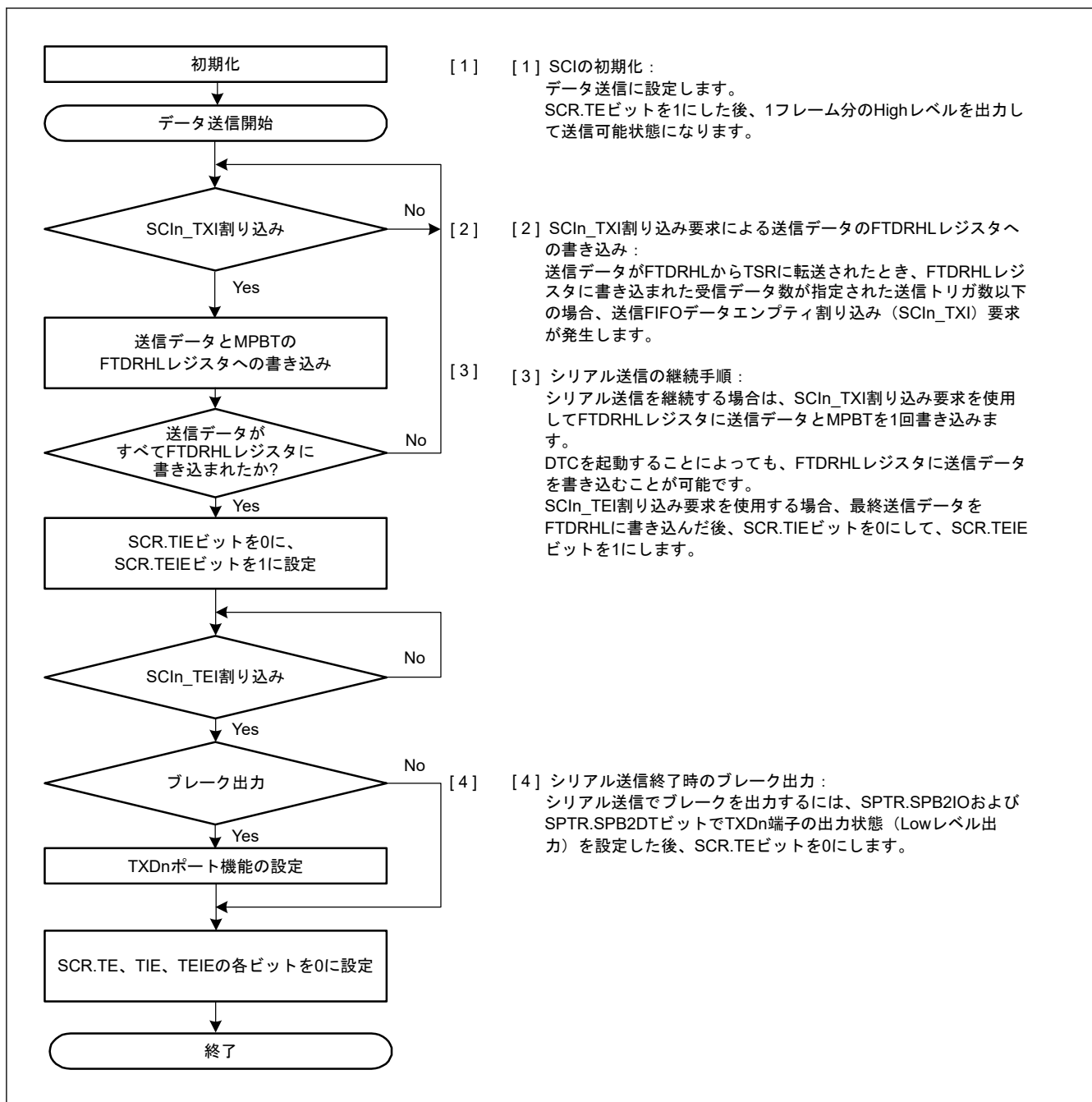
図 24.27 マルチプロセッサシリアル送信のフローチャート例（非 FIFO 選択時）
