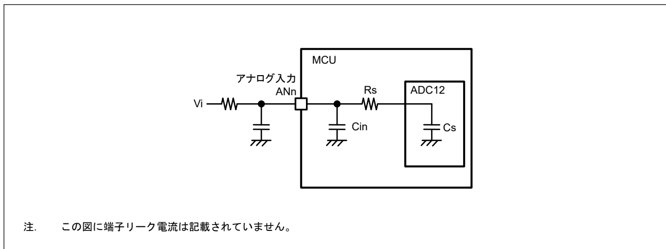
図 35.49 アナログ入力の等価回路
