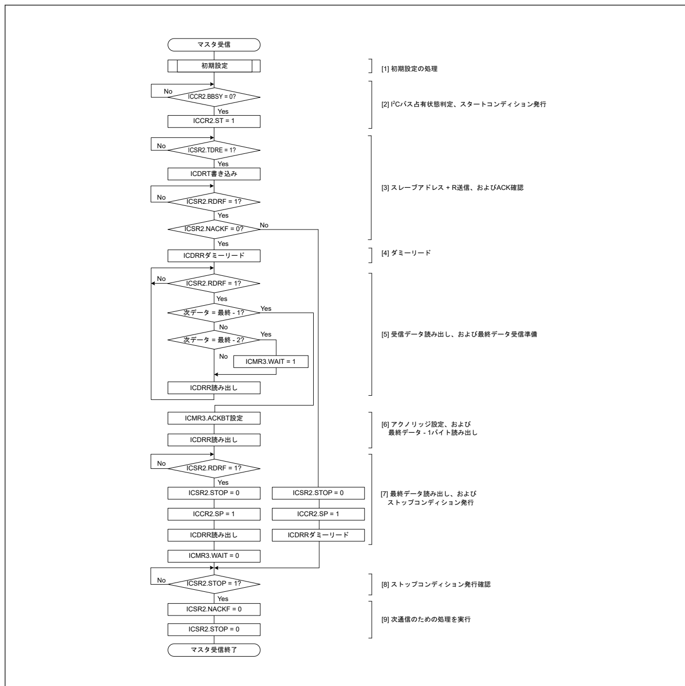
図 25.11 マスタ受信の例 (7 ビットアドレスフォーマットで 3 バイト以上受信の場合)
