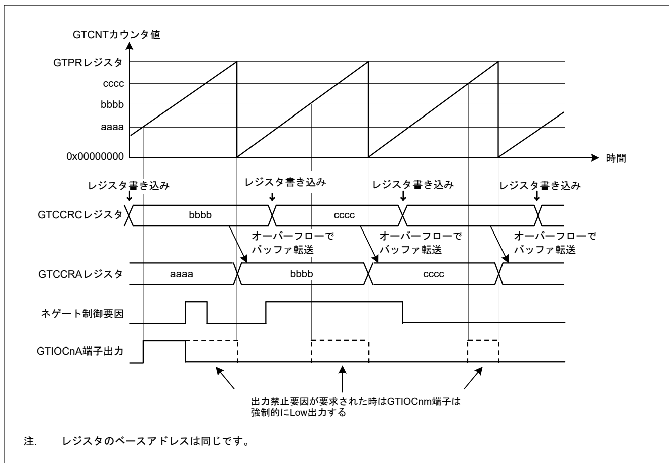
図 20.170 GTIOcnm 端子出力禁止制御の動作例（のこぎり波でアップカウント、バッファ動作、アクティブレベル 1、GTCCRA レジスタのコンペアマッチで High 出力、周期の終わりで Low 出力、出力禁止で Low 出力の場合）（ n = 0 \sim 3 , m = A, B ）
