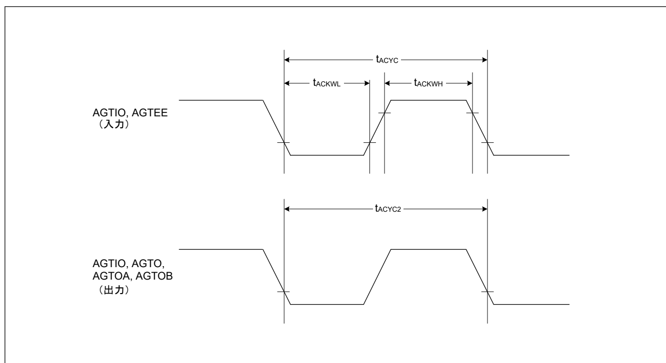
図 35.28 AGTW I/O タイミング
