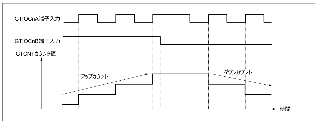
図 20.125 位相計数モード2の動作例 (B)
