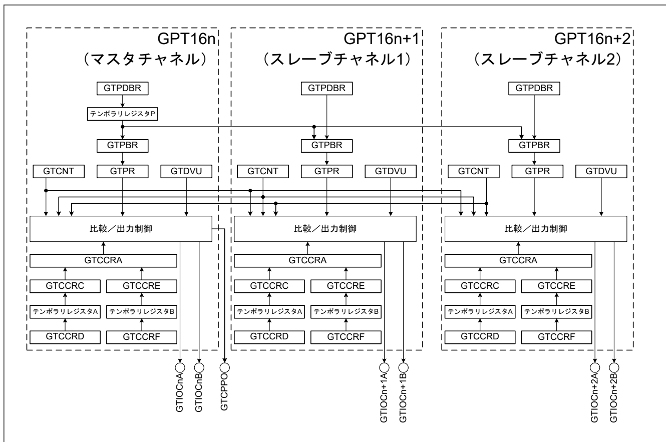
図 20.46 相補 PWM モード 1、2、3 のブロック図 ( n = 0 )
