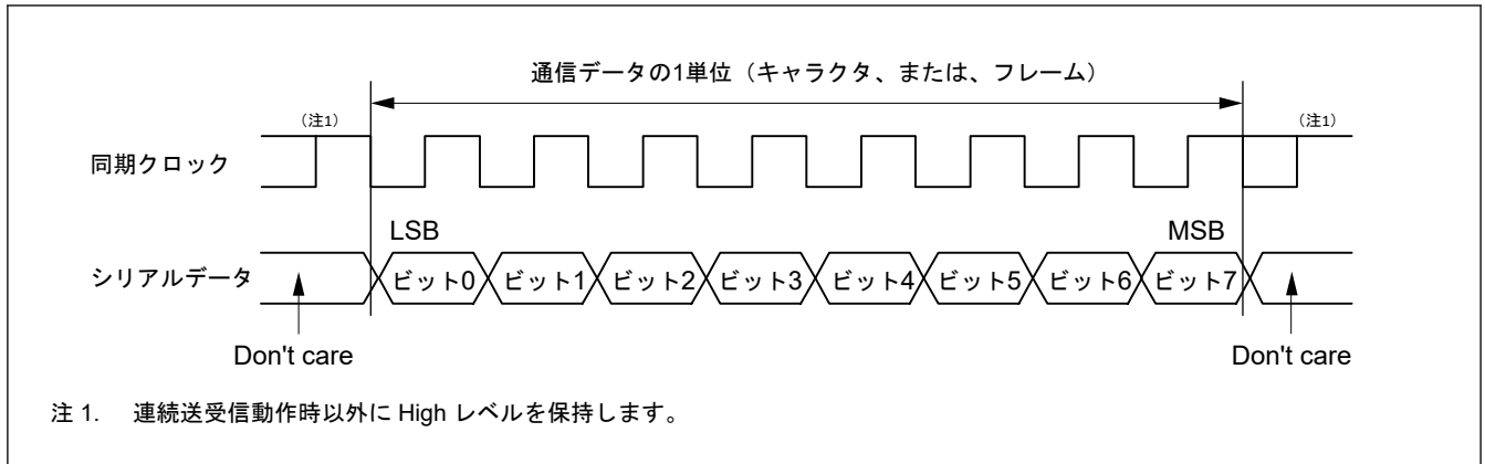
図 24.35 クロック同期式シリアル通信のデータフォーマット（LSB ファーストの並び順の場合）
