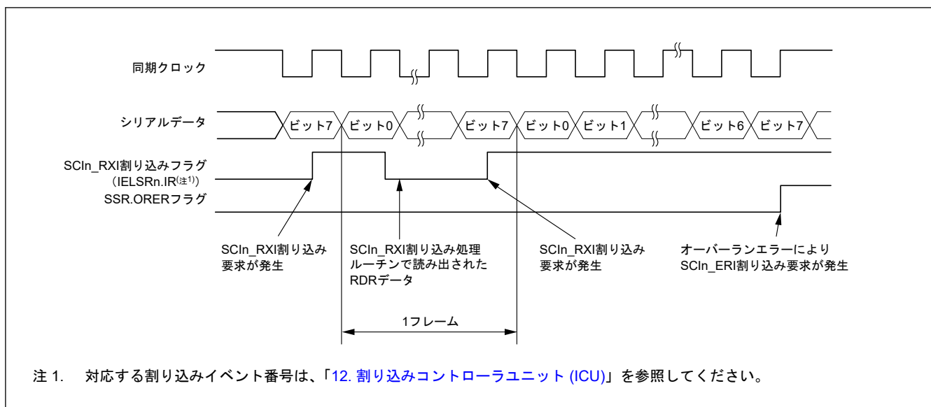
図 24.41 クロック同期式モードにおけるシリアル受信の動作例 (1) (RTS 機能を使用しない場合)
