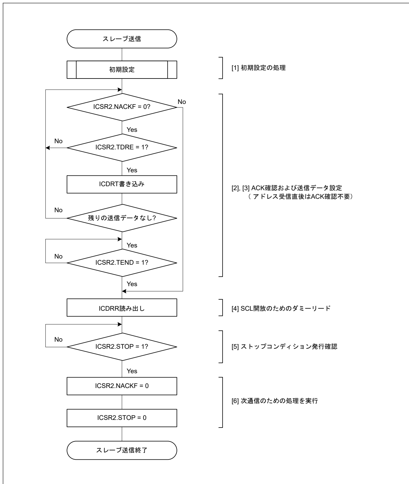
図 25.15 スレーブ送信のフローチャート例
