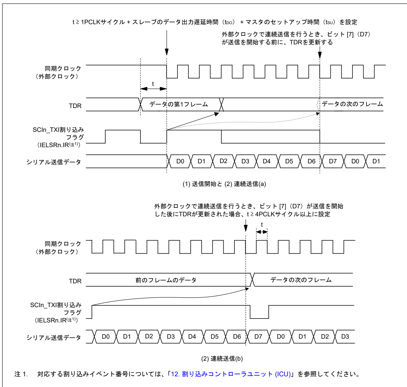
図 24.77 クロック同期式送信時の外部クロック使用に関する制約事項
