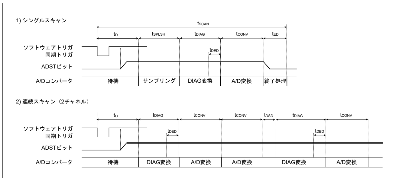
図 29.29 スキャン変換のタイミング (ソフトウェア起動または同期トリガ入力 (ELC) 起動の場合)
