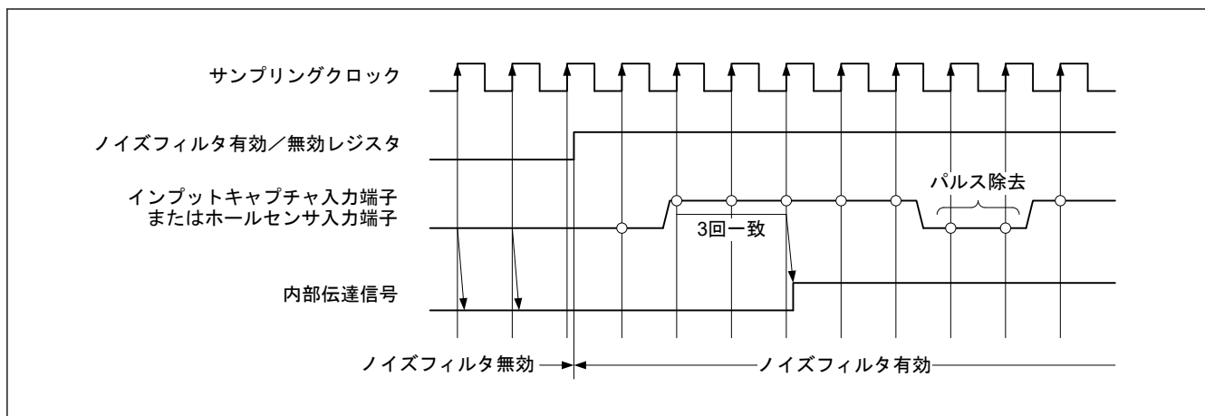
図 20.162 ノイズフィルタのタイミング
