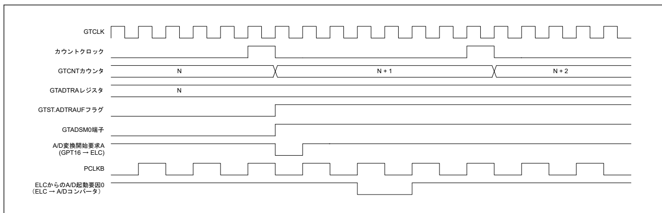
図 20.161 A/D 変換開始要求タイミング動作例
