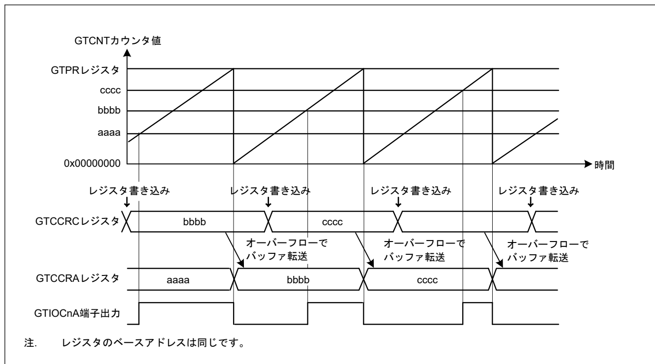
図 20.24 GTCCRA および GTCCRB レジスタのバッファ動作例 (アウトプットコンペア、アップカウント時ののこぎり波 PWM モード 1、GTCCRA レジスタのコンペアマッチで High 出力、周期の終わりで Low 出力の場合)
