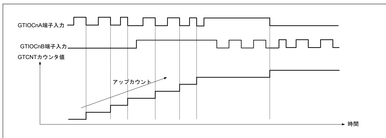
図 20.131 位相計数モード 5 の動作例 (A)
