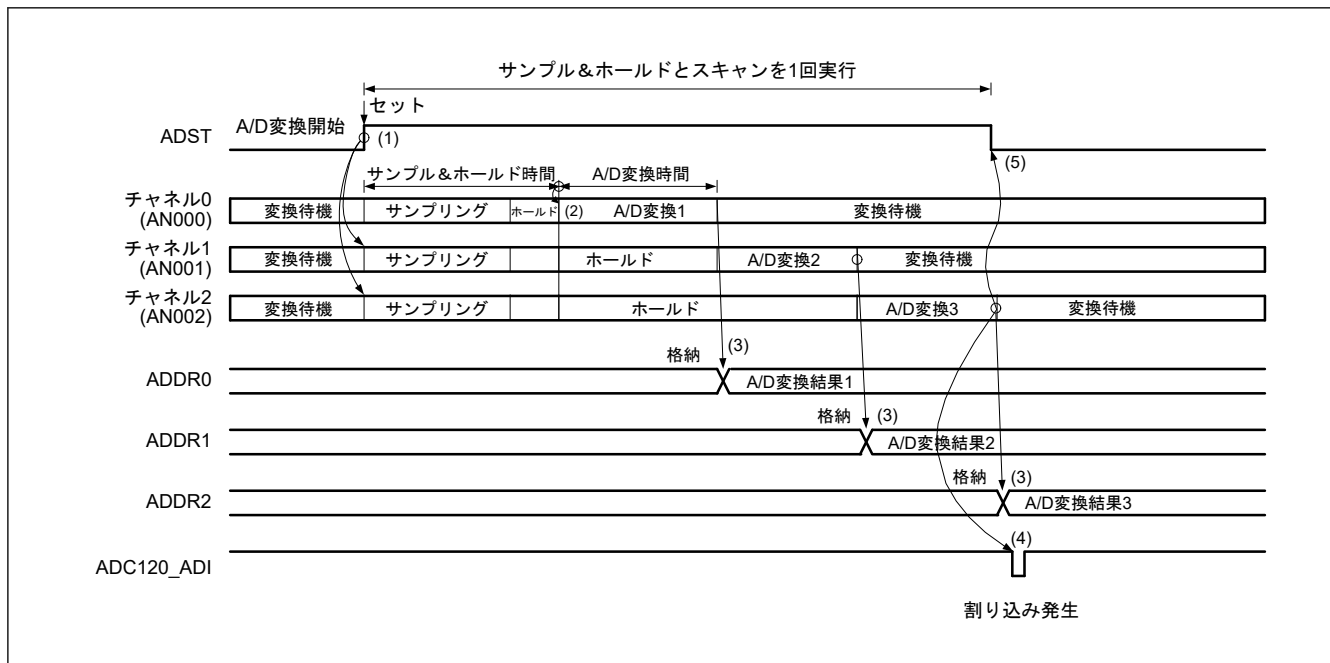
図 29.8 シングルスキャンモードの動作例（チャンネル専用サンプル&ホールド回路使用、AN000～AN002 選択）
