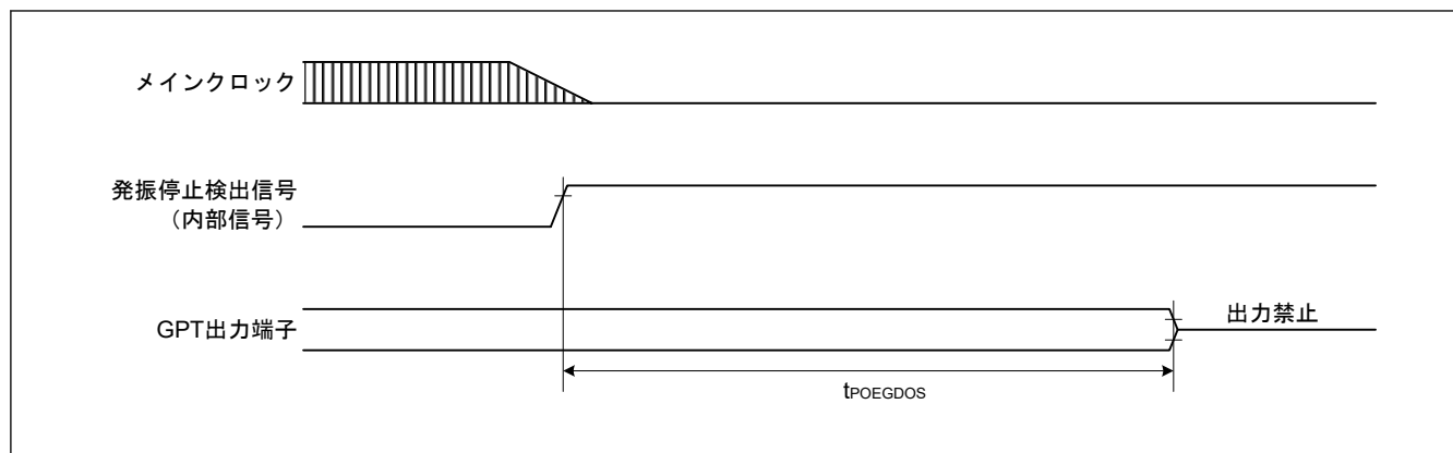
図 35.19 発振停止検出に対応した POEG の出力禁止時間
