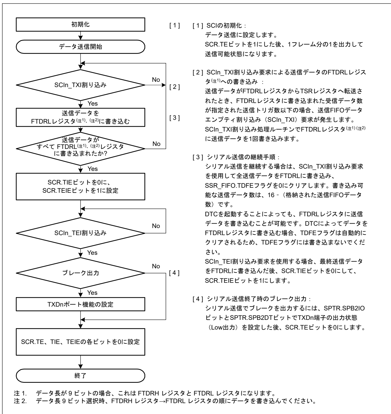
図 24.12 調歩同期式モードにおけるシリアル送信のフローチャート例（FIFO 選択時）
