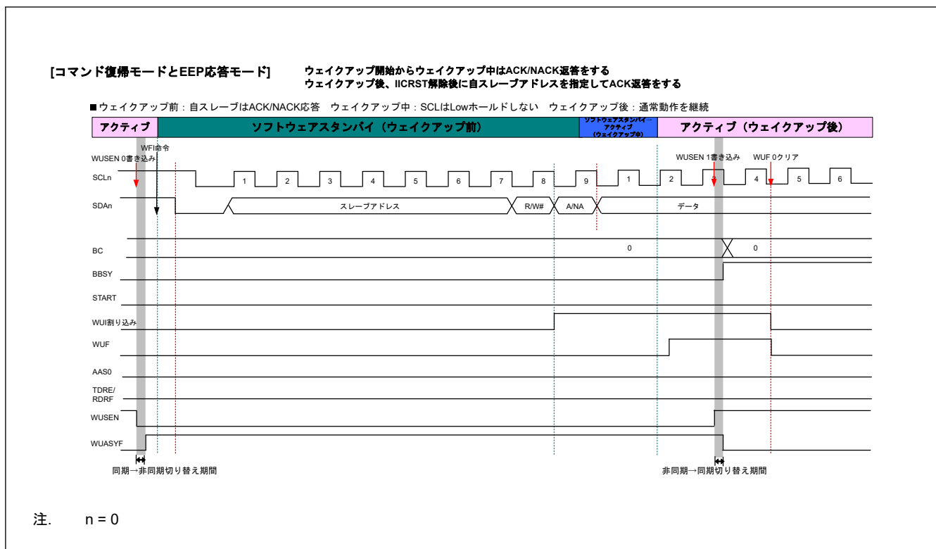
図 25.37 コマンドリカバリモードとEEP 応答モードのタイミング
