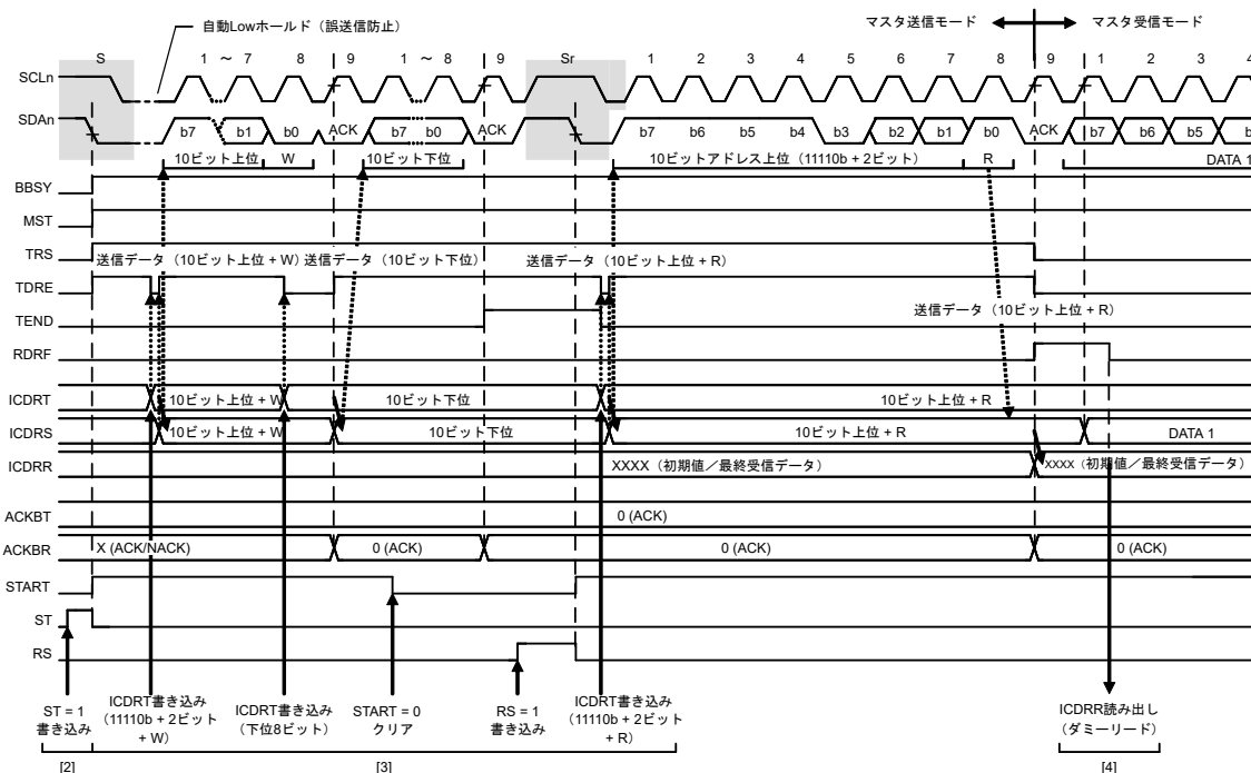
図 25.13 マスタ受信の動作タイミング (2) (10 ビットアドレスフォーマットで RDRFS = 0 の場合)
