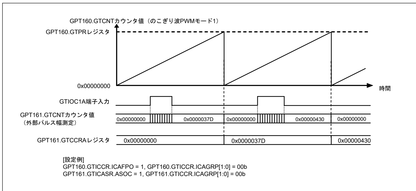
図 20.114 チャンネル間連携によるインプットキャプチャ動作例 (チャンネル 0 のオーバーフローでチャンネル 1 をキャプチャ)
