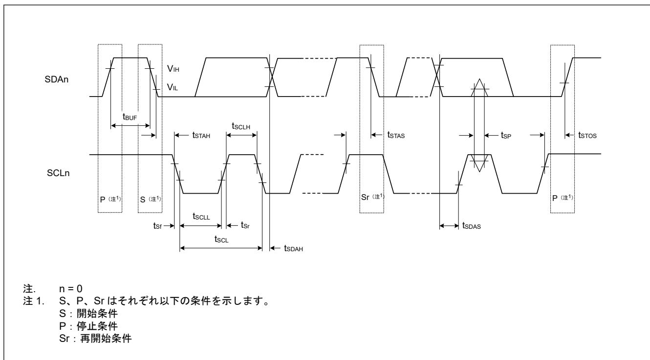
図 35.46 I 2 C バスインタフェース入出力タイミング
