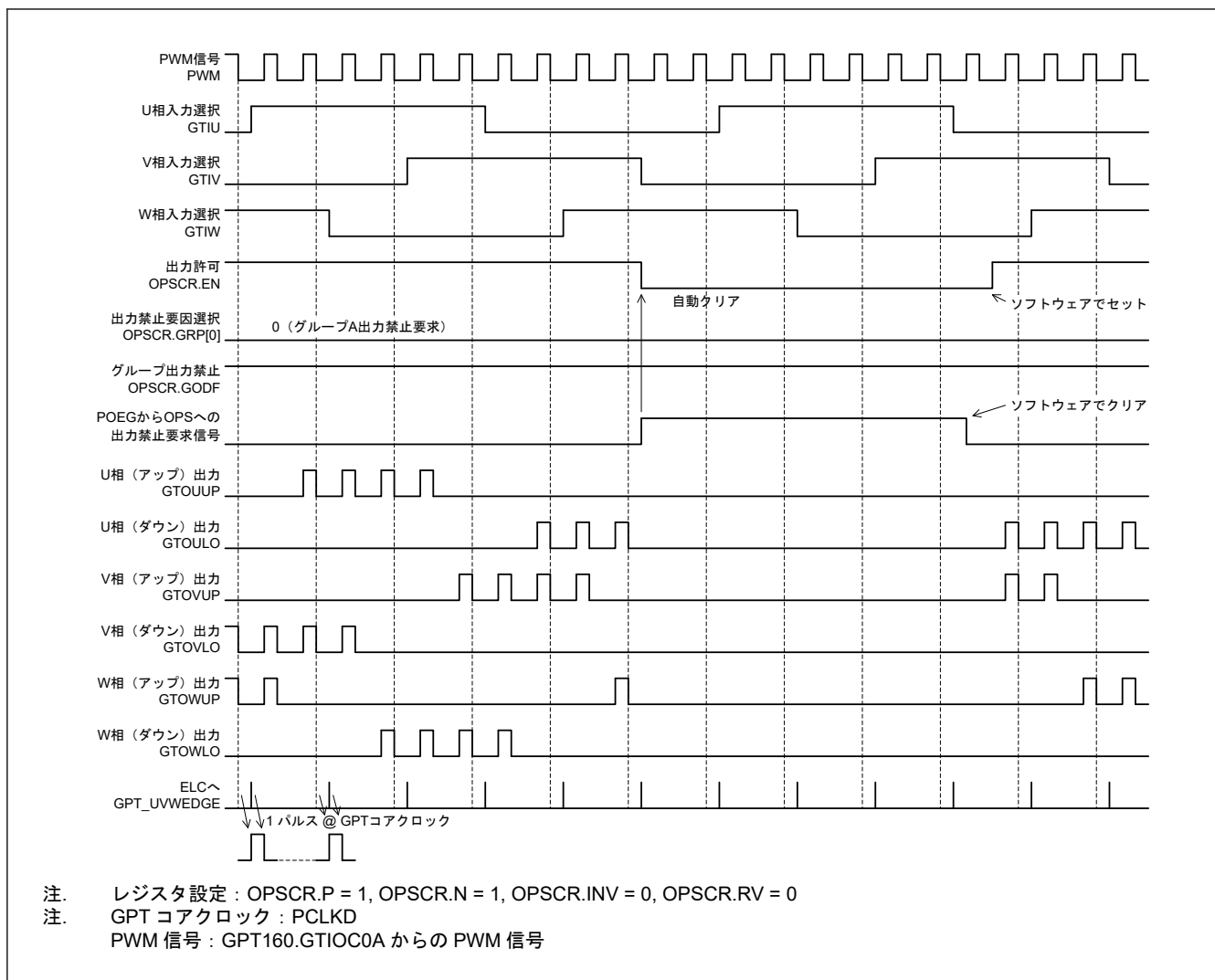
図 20.138 グループ出力禁止制御動作例
