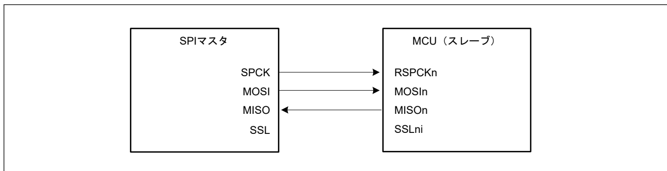
図 26.11 クロック同期式動作のマスタとスレーブの構成例 (MCU はスレーブ、CPHA = 1)
