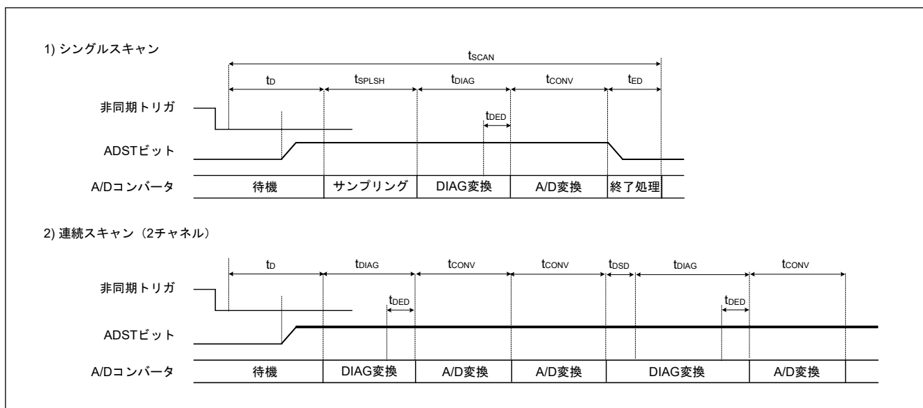
図 29.30 スキャン変換のタイミング (非同期トリガ入力 (ADTRG0) 起動の場合)
