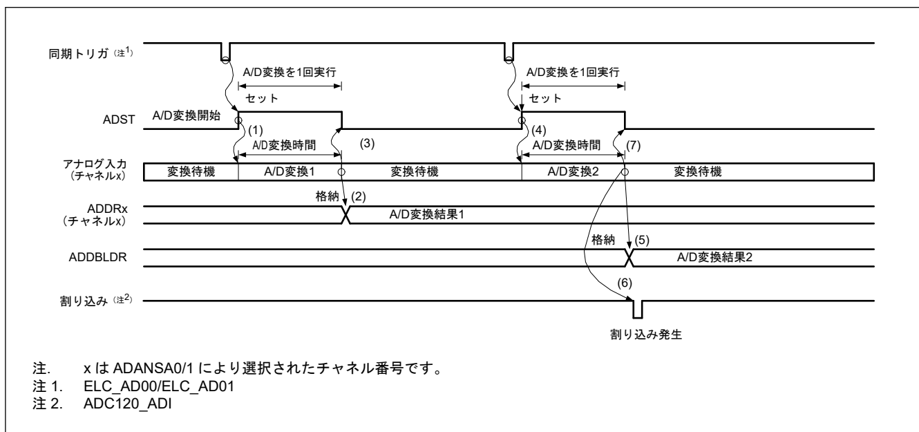
図 29.12 シングルスキャンモードの動作例 (ダブルトリガモード選択、アナログ入力 (チャンネル x) を 2 重化)
