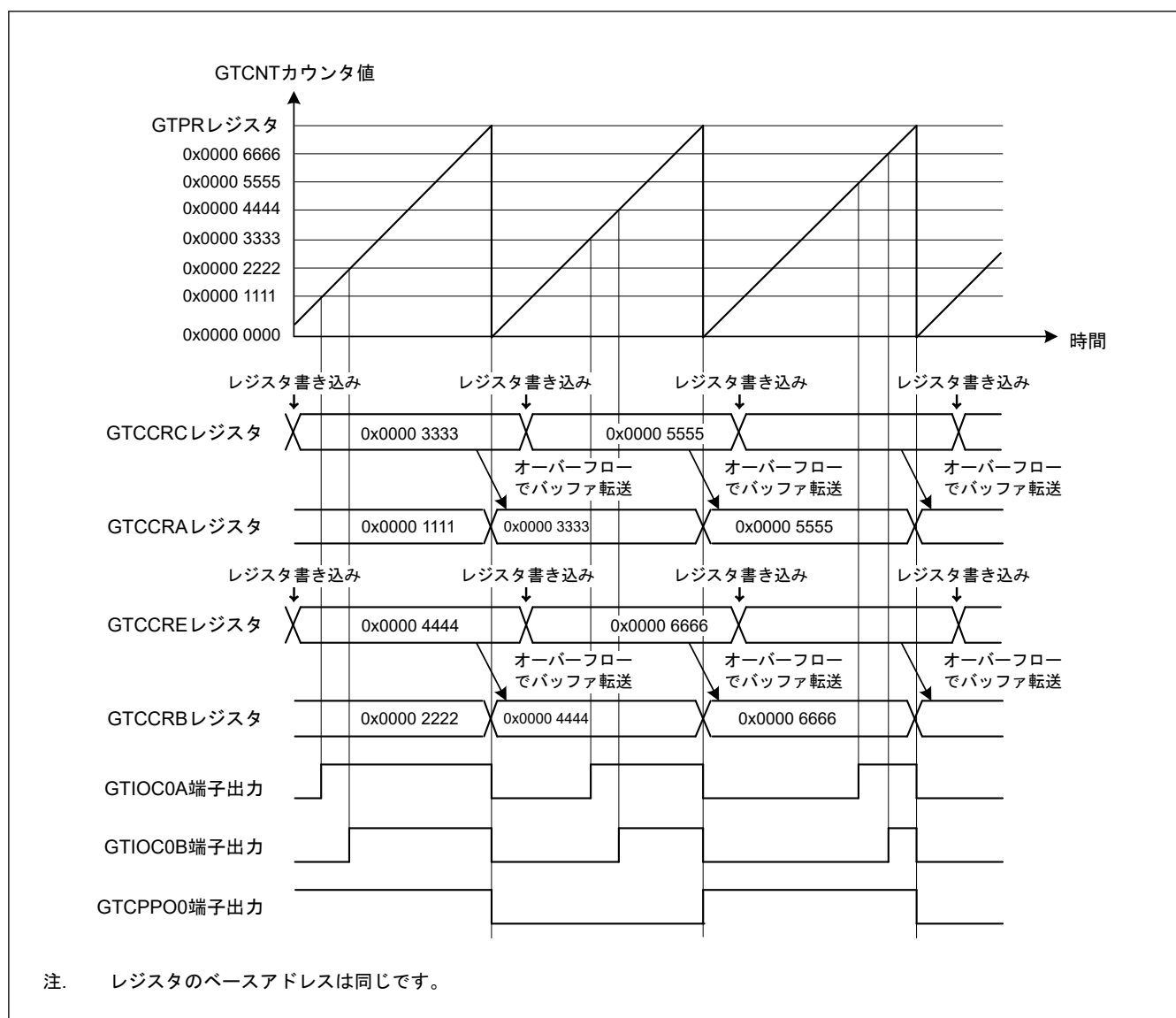
図 20.38 のこぎり波 PWM モード 1 の動作例 (アップカウント、バッファ動作、GTCCR/GTCCR レジスタのコンペアマッチで High 出力、周期の終わりで Low 出力、GTIOR.PSYE = 1 の場合)
