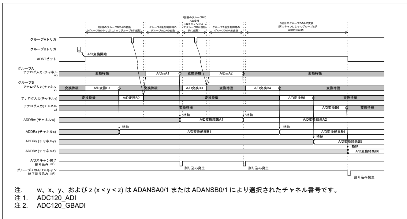
図 29.22 グループ優先動作の例 1-2 : グループ B 再スキャン中のグループ A トリガ入力、再スキャンあり (ADGSPCR.GBRSCN = 1、ADGSPCR.GBRP = 0 の場合)
