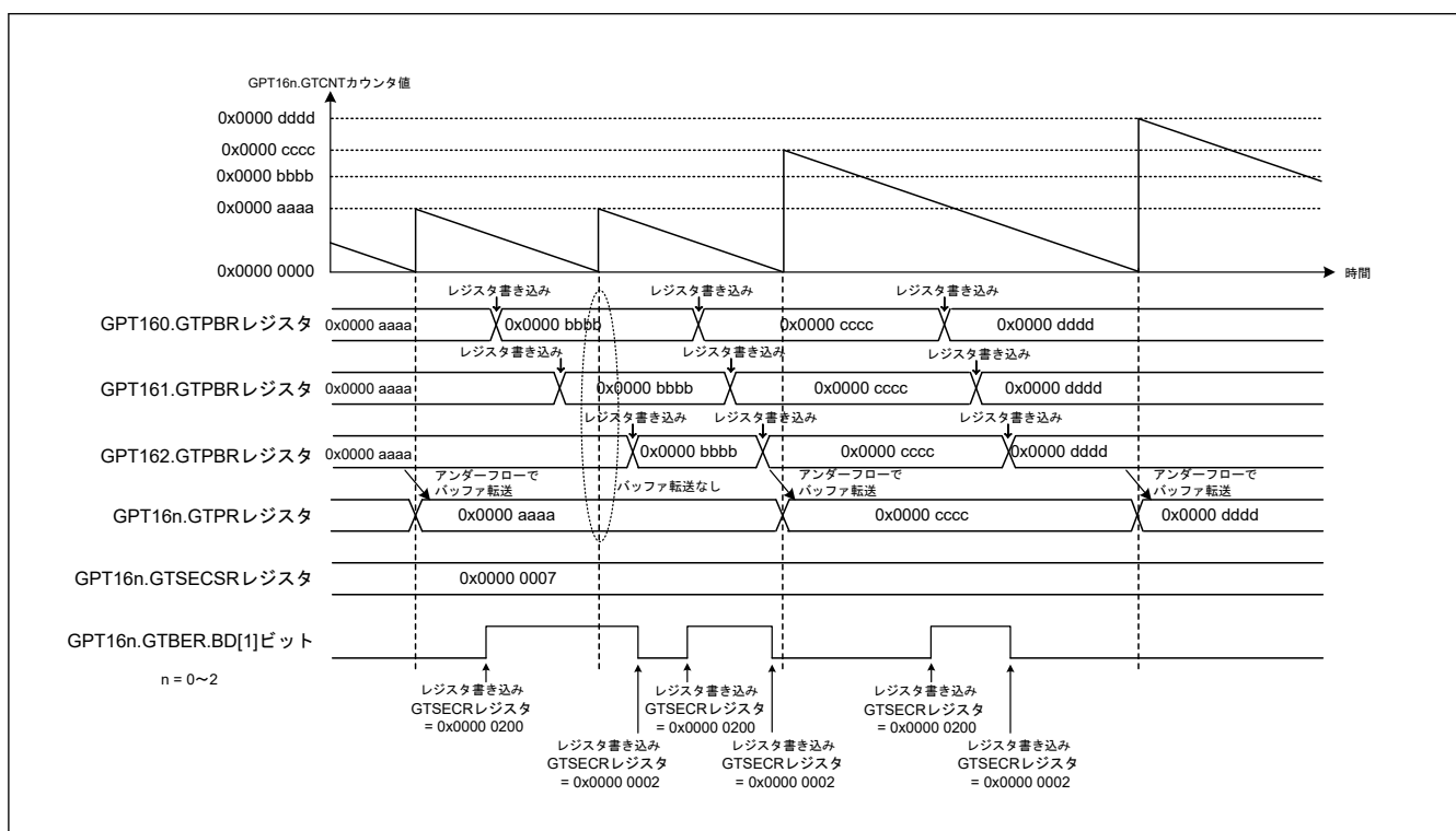
図 20.165 バッファ動作禁止の複数チャネルの動作例 (のこぎり波、シングルバッファ動作)
