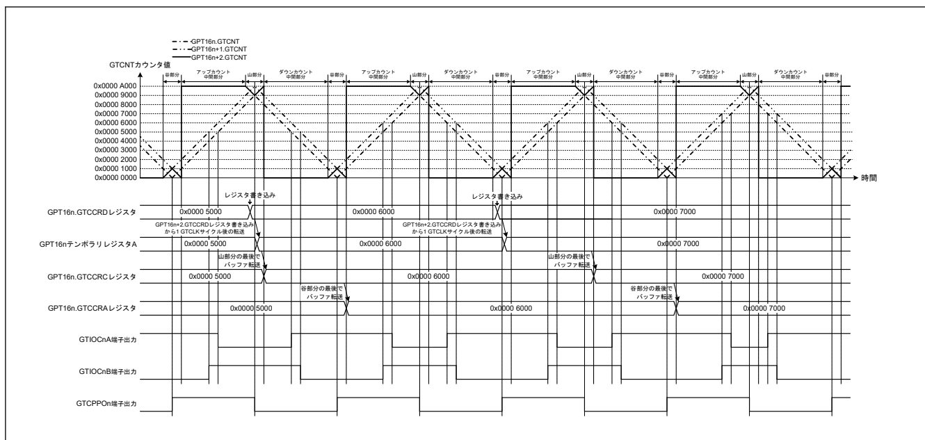
図 20.50 相補 PWM モード 2 動作例 (アップカウントの GTCCRA レジスタコンペアマッチ時: GTIOCnA 端子 = Low/GTIOCnB 端子 = High、ダウンカウントの GTCCRA レジスタコンペアマッチ時: GTIOCnA 端子 = High/GTIOCnB 端子 = Low、デッドタイム値: 0x0000 1000、GTCCRD レジスタを山部分と谷部分で更新) (n = 0)
