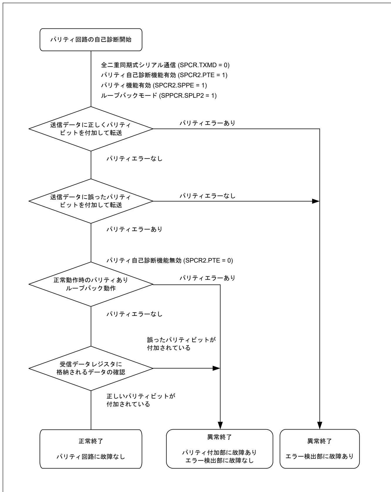
図 26.42 パリティ回路の自己診断フロー
