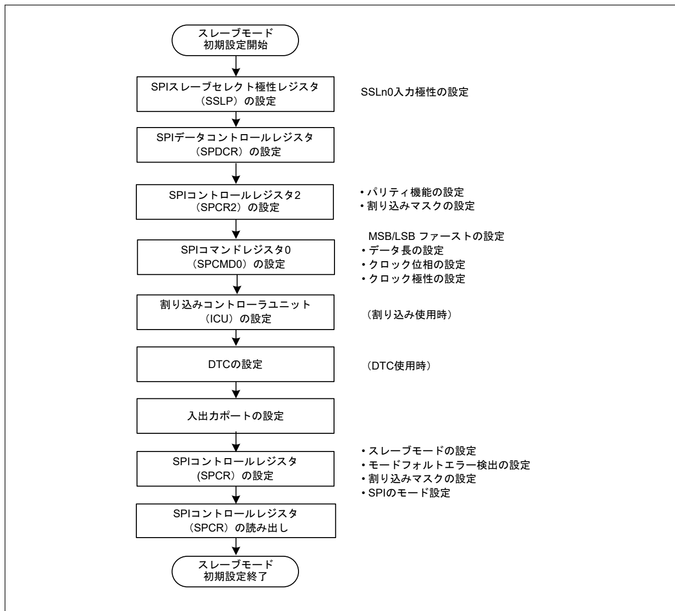
図 26.35 スレープモード時の SPI 動作の初期化フロー例
