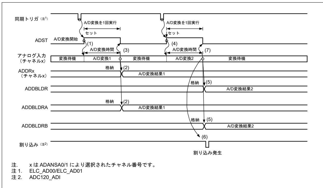
図 29.13 アナログ入力 (チャンネル x) と ELC_AD00/ELC_AD01 の重複選択時のダブルトリガモード拡張動作例
