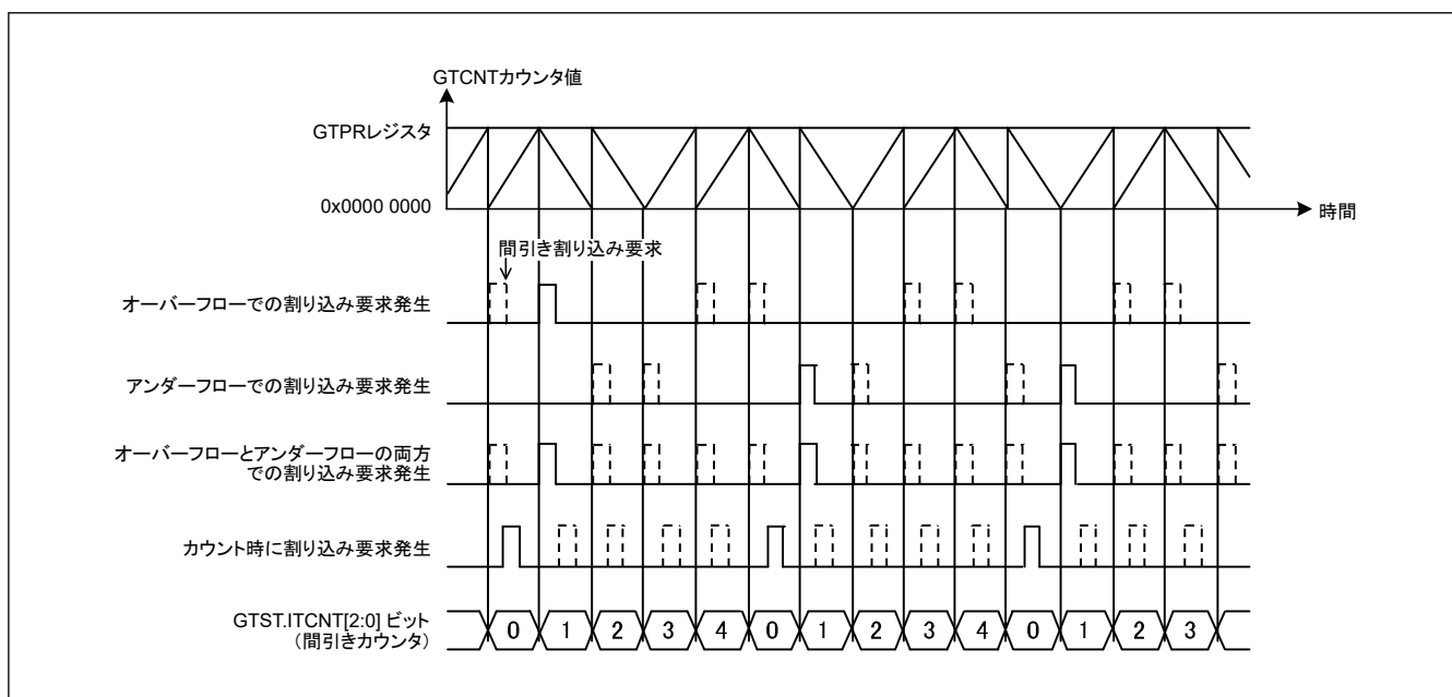
図 20.144 割り込み間引き機能の動作例（のこぎり波でカウント方向を変えながら動作、オーバーフローとアンダーフローの両方をカウントして間引き、間引き回数 4 の場合）
