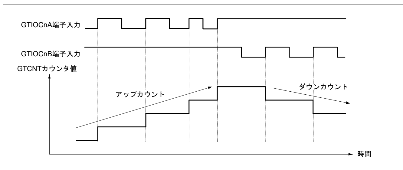
図 20.128 位相計数モード3の動作例 (B)
