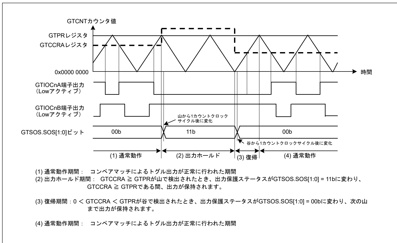
図 20.179 山でのバッファ転送中に GTCCR \geq GTPR となったときの出力保護機能の動作例（谷でのバッファ転送中に 0 < GTCCR < GTPR に復帰、アクティブレベル：Low）（ n = 0 \sim 2 ）
