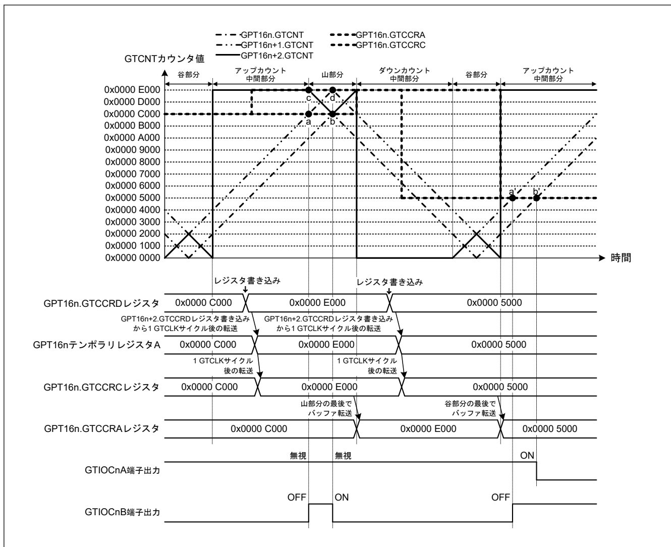
図 20.58 相補 PWM モードでのコンペアマッチ発生シーケンス動作例 (相補 PWM モード 3 シングルバッファ動作、アップカウントの GTCCRA レジスタコンペアマッチ時: GTIOcNA 端子 = Low/GTIOcNB 端子 = High、ダウンカウントの GTCCRA レジスタコンペアマッチ時: GTIOcNA 端子 = High/GTIOcNB 端子 = Low、デッドタイム値: 0x0000 2000、コンペアマッチ発生順序: (a, c) → (b, d)) (n = 0)
