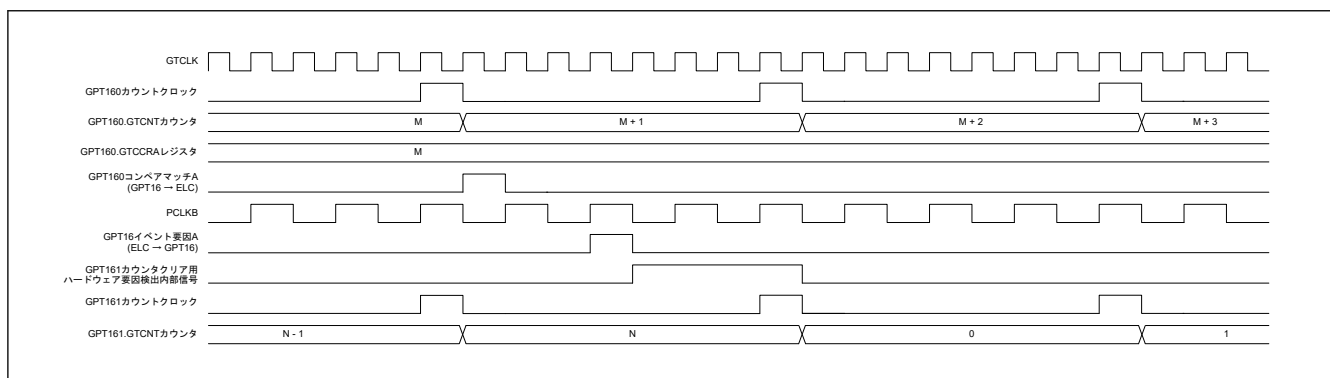
図 20.103 ELC_GPTA からのイベント入力に対応するカウンタクリアの動作タイミング例 (GTCLK 信号の分周により生成されるクロック信号の周期計数中)
