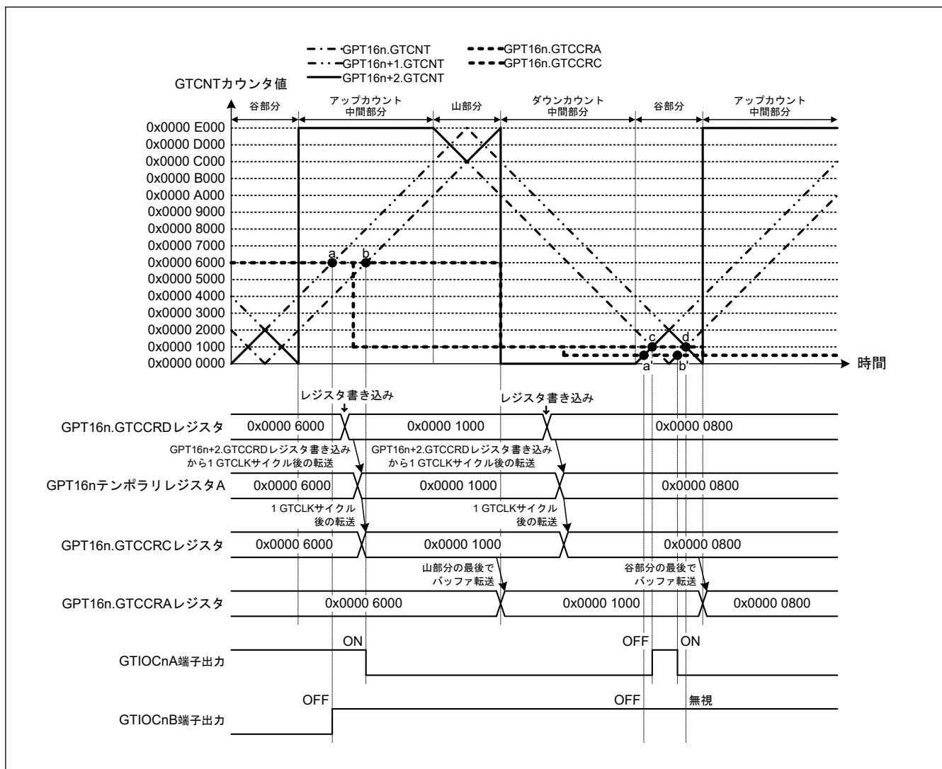
図 20.65 相補 PWM モードでのコンペアマッチ発生シーケンス動作例 (相補 PWM モード 3 シングルバッファ動作、アップカウントの GTCCRA レジスタコンペアマッチ時: GTIOCnA 端子 = Low/GTIOCnB 端子 = High、ダウンカウントの GTCCRA レジスタコンペアマッチ時: GTIOCnA 端子 = High/GTIOCnB 端子 = Low、デッドタイム値: 0x0000 2000、コンペアマッチ発生順序: a' → c → b' → d) (n = 0)
