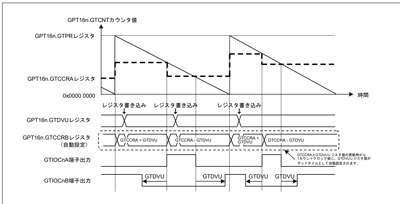
図 20.82 デッドタイム自動設定機能の動作例 (のこぎり波ワンショットパルスモード、ダウンカウント、GPT163 でアクティブ High の場合)
