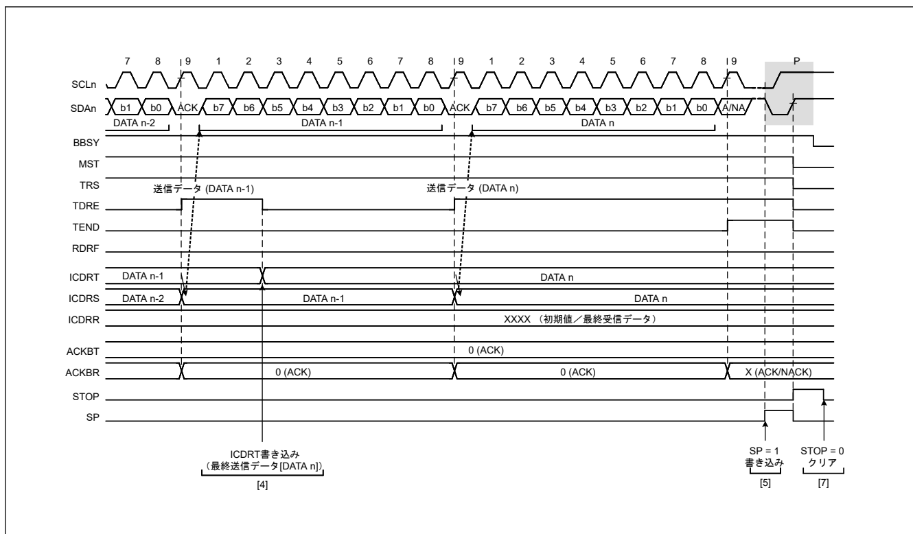
図 25.9 マスタ送信の動作タイミング (3)
