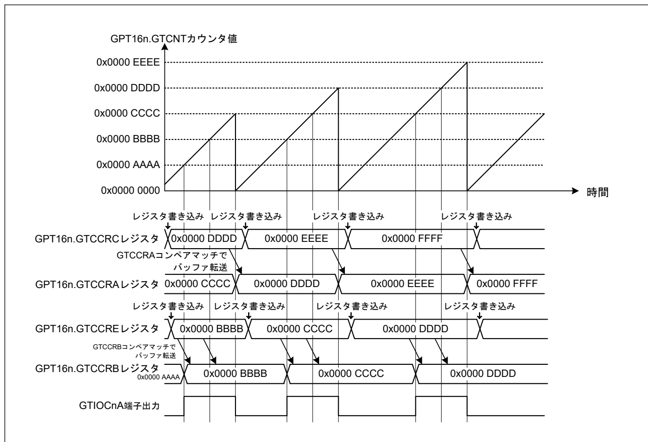
図 20.25 GTCCRA および GTCCRB レジスタのバッファ動作例（アウトプットコンペア、のこぎり波 PWM モード 2、GTCCRA レジスタのコンペアマッチでのバッファ転送、カウンタクリア、Low 出力、GTCCRB レジスタのコンペアマッチでのバッファ転送、High 出力）（n = 0~2）
