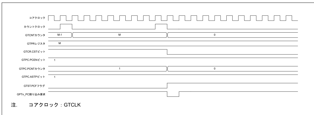
図 20.122 PWM 周期計数機能の動作タイミング例 (のこぎり波ワンショットパルスモード、アップカウント)
