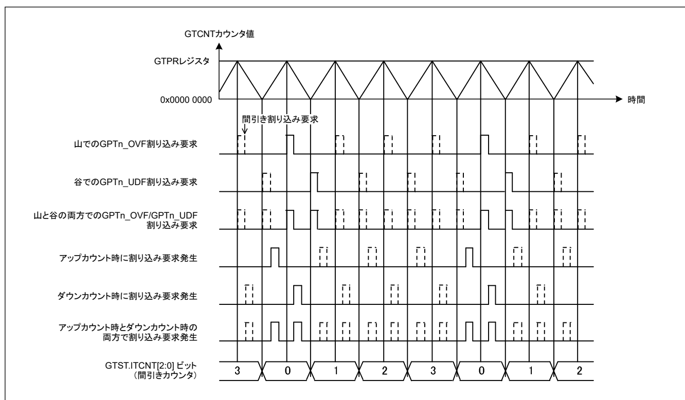
図 20.140 割り込み間引き機能の動作例（三角波、谷をカウントして間引き、間引き回数 3 の場合）
