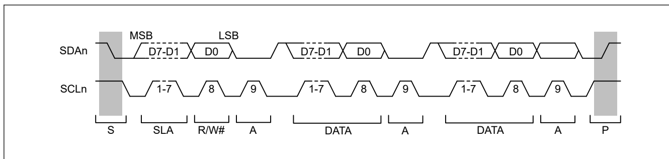
図 24.59 I 2 C バスタイミング (SLA = 7 ビットの場合)
