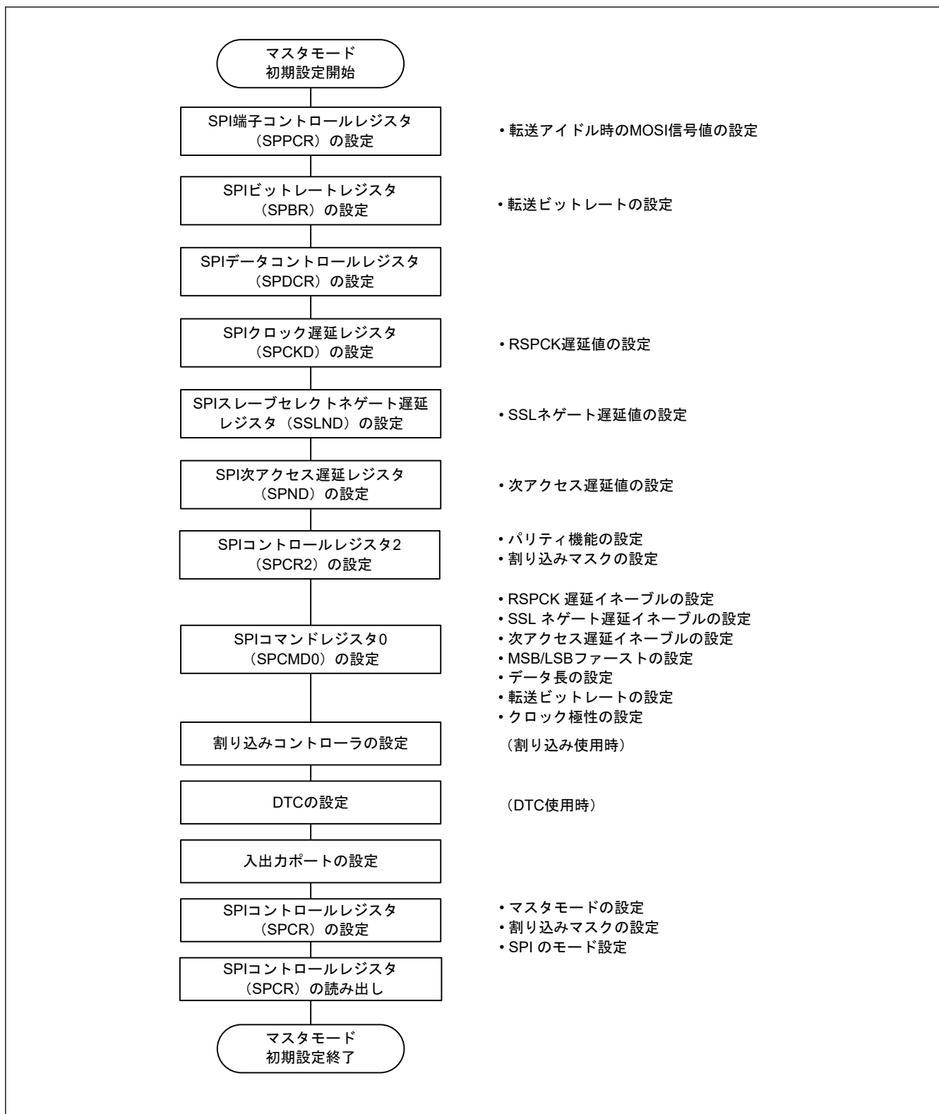
図 26.39 マスタモード時のクロック同期式動作の初期化フロー例
