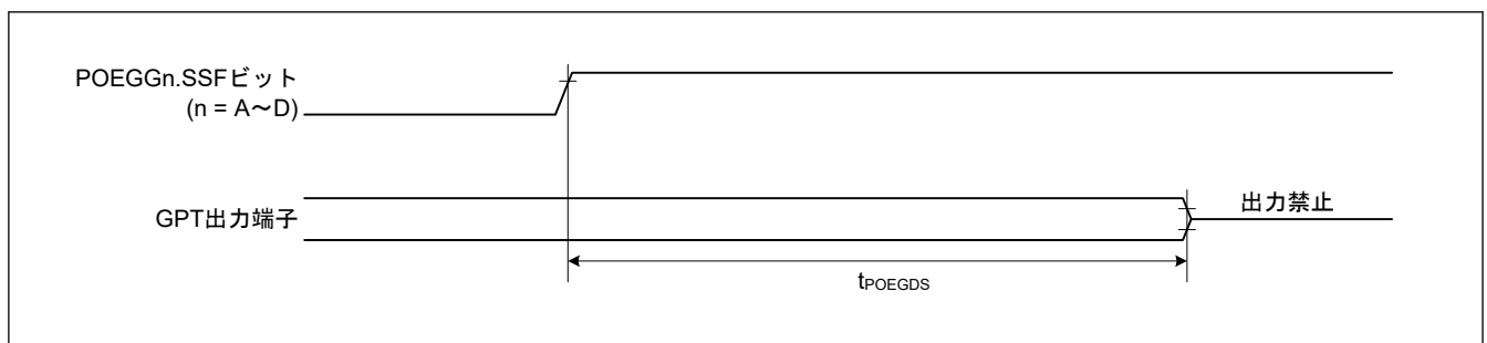
図 35.18 レジスタ設定に対応した POEG の出力禁止時間
