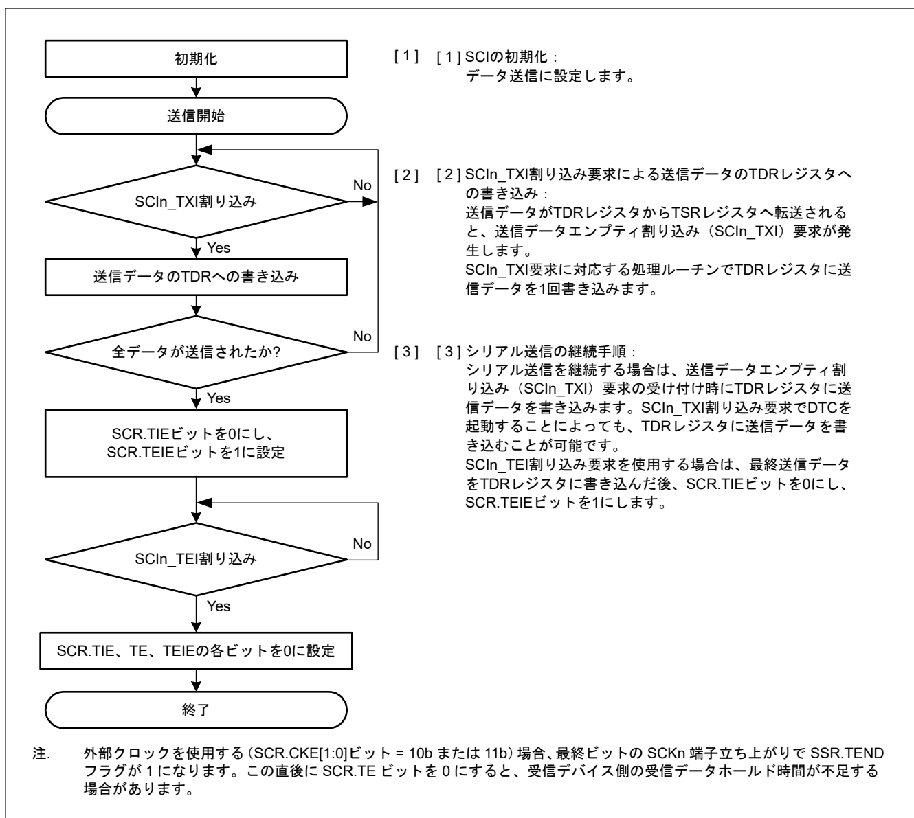
図 24.39 クロック同期式モードにおけるシリアル送信のフローチャート例 (非 FIFO 選択時)
