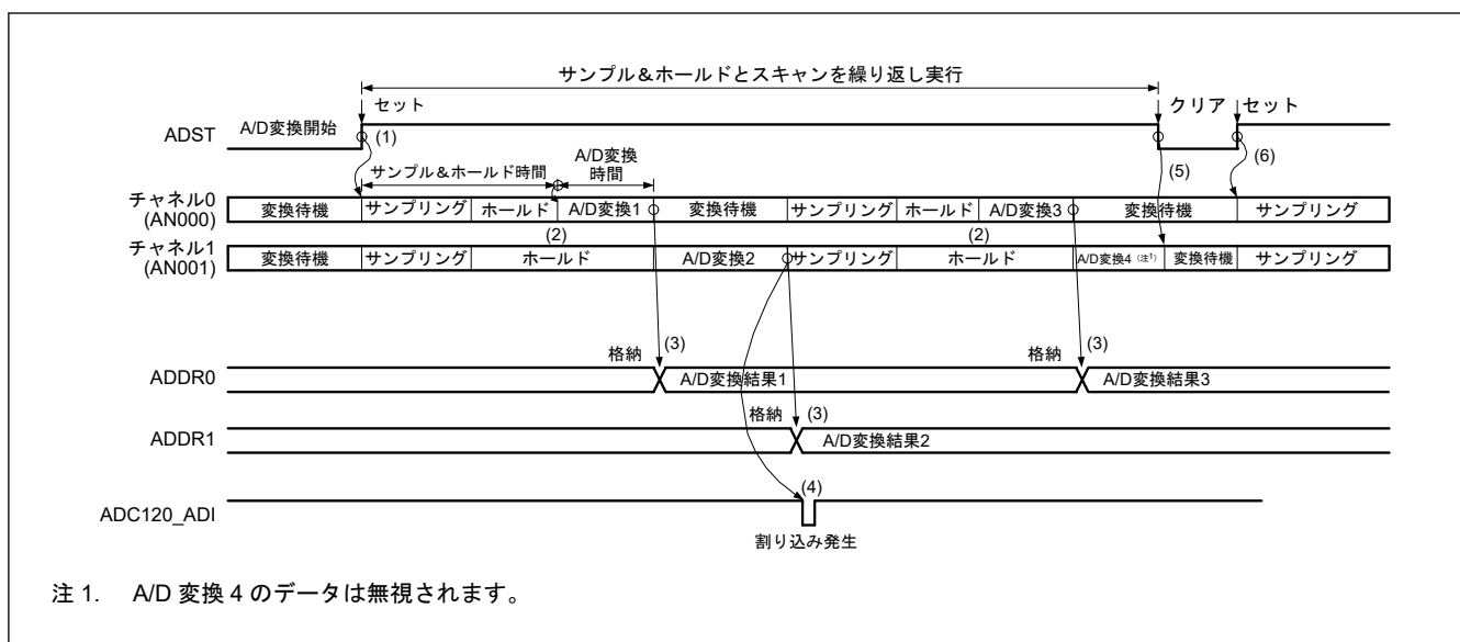
図 29.15 連続スキャンモードの動作例 (チャンネル専用サンプル&ホールド回路使用、AN000 および AN001 選択)
