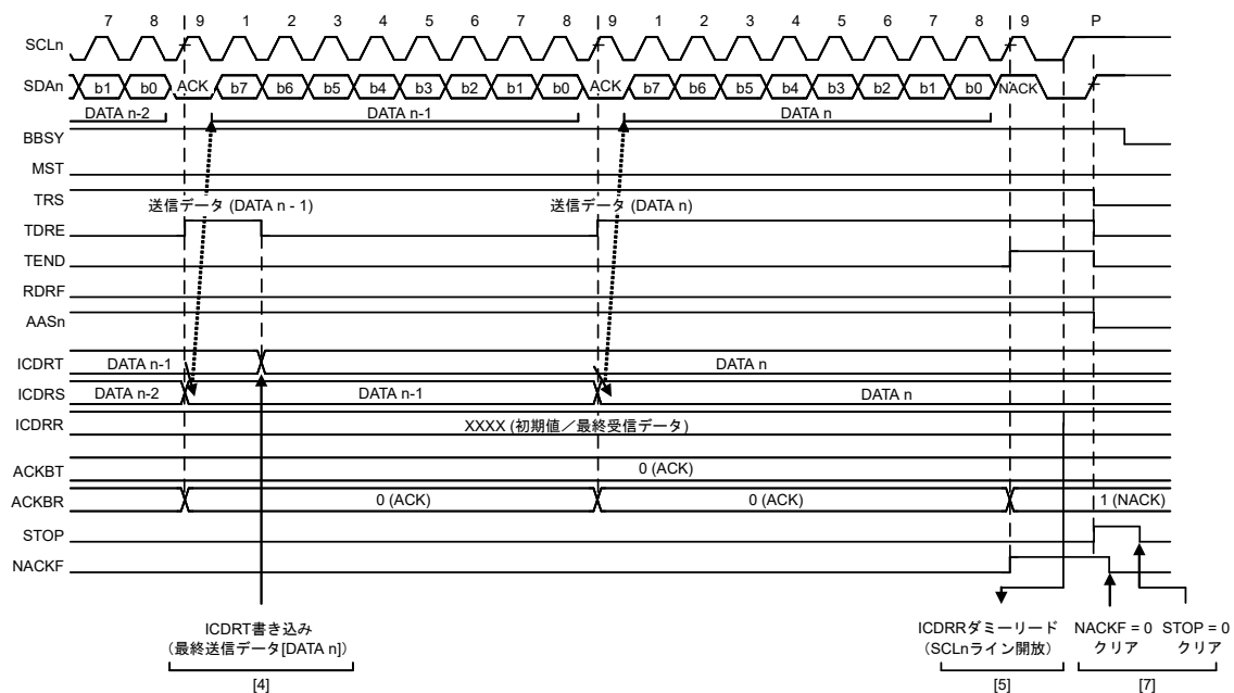
図 25.17 スleep送信の動作タイミング (2)
