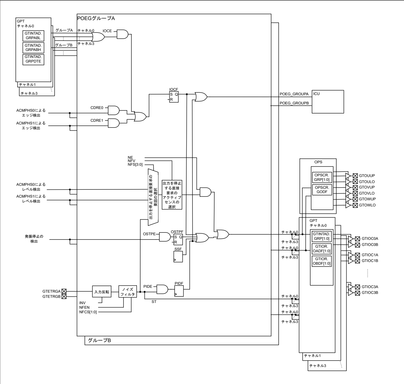
図 19.1 POEG のブロック図
