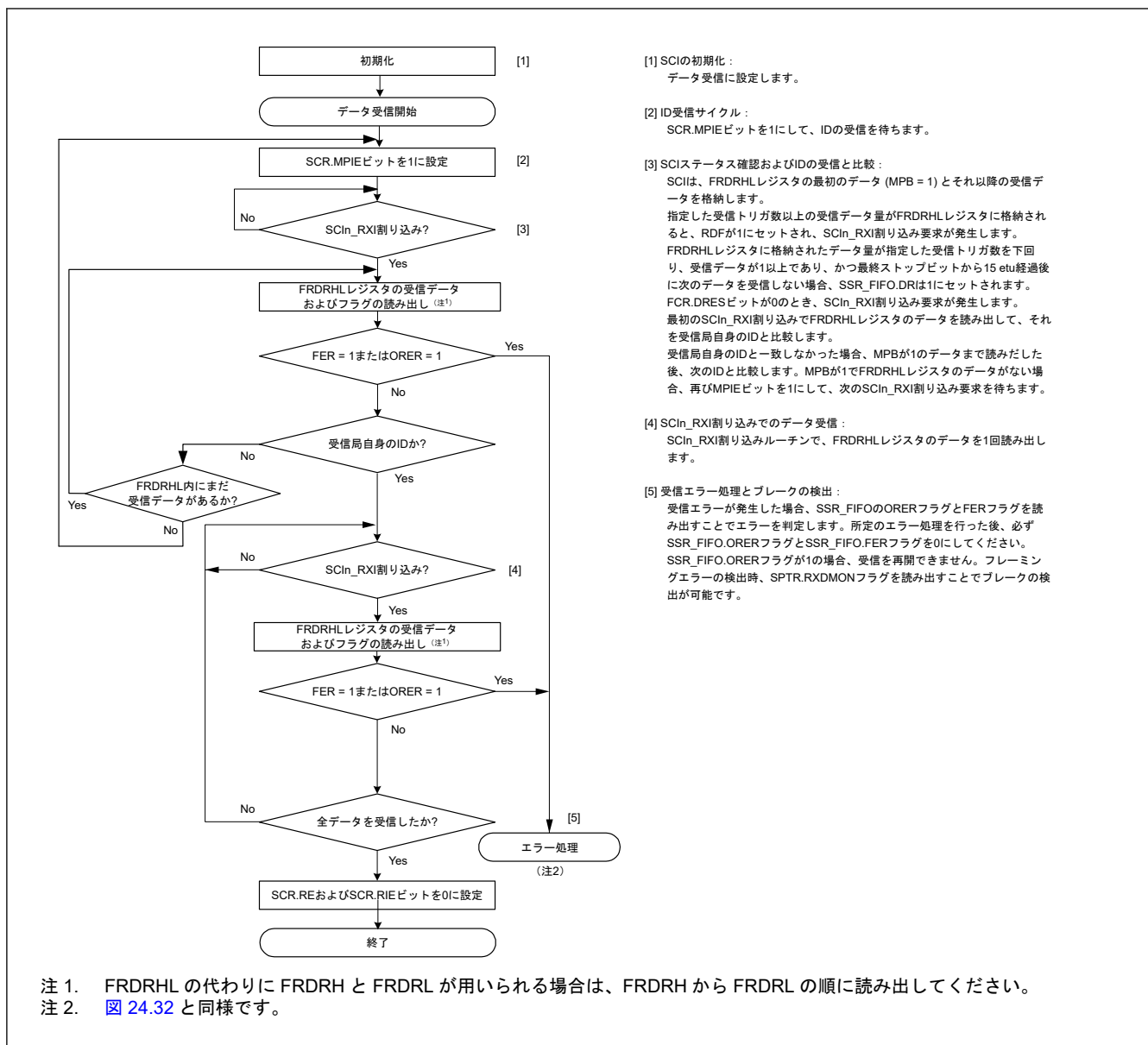
図 24.34 マルチプロセッサモードにおけるシリアル受信のフローチャート例 (FIFO 選択時)
