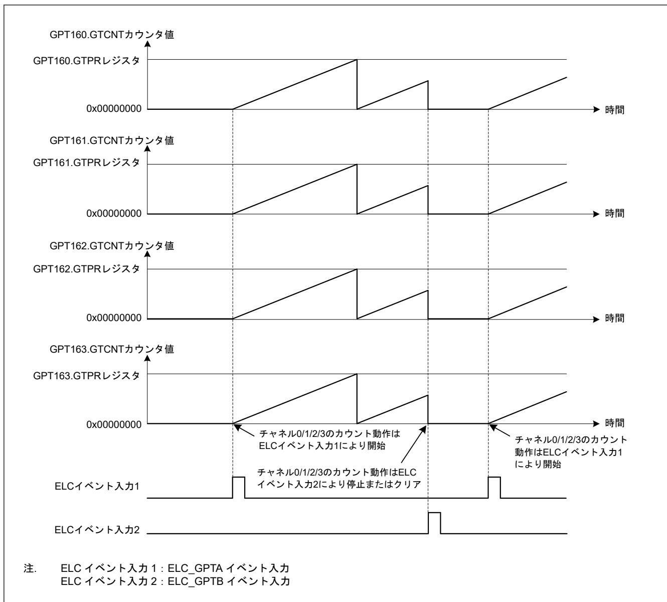
図 20.112 ハードウェア要因による同時スタート/ストップ/クリア動作例 (カウント周期 (GTPR レジスタ値) が同一のとき)
