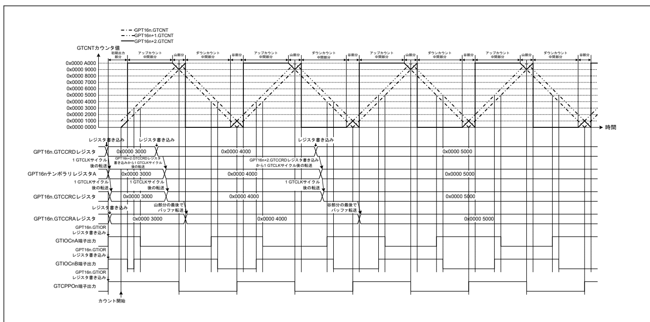
図 20.51 相補 PWM モード 3 動作例 (シングルバッファ動作、初期出力時: GTIOCnA 端子 = High/GTIOCnB 端子 = High、アップカウントの GTCCRA レジスタコンペアマッチ時: GTIOCnA 端子 = Low/GTIOCnB 端子 = High、ダウンカウントの GTCCRA レジスタコンペアマッチ時: GTIOCnA 端子 = High/GTIOCnB 端子 = Low、デッドタイム値: 0x0000 1000、GTCCRD レジスタを中間部分で更新) (n = 0)
