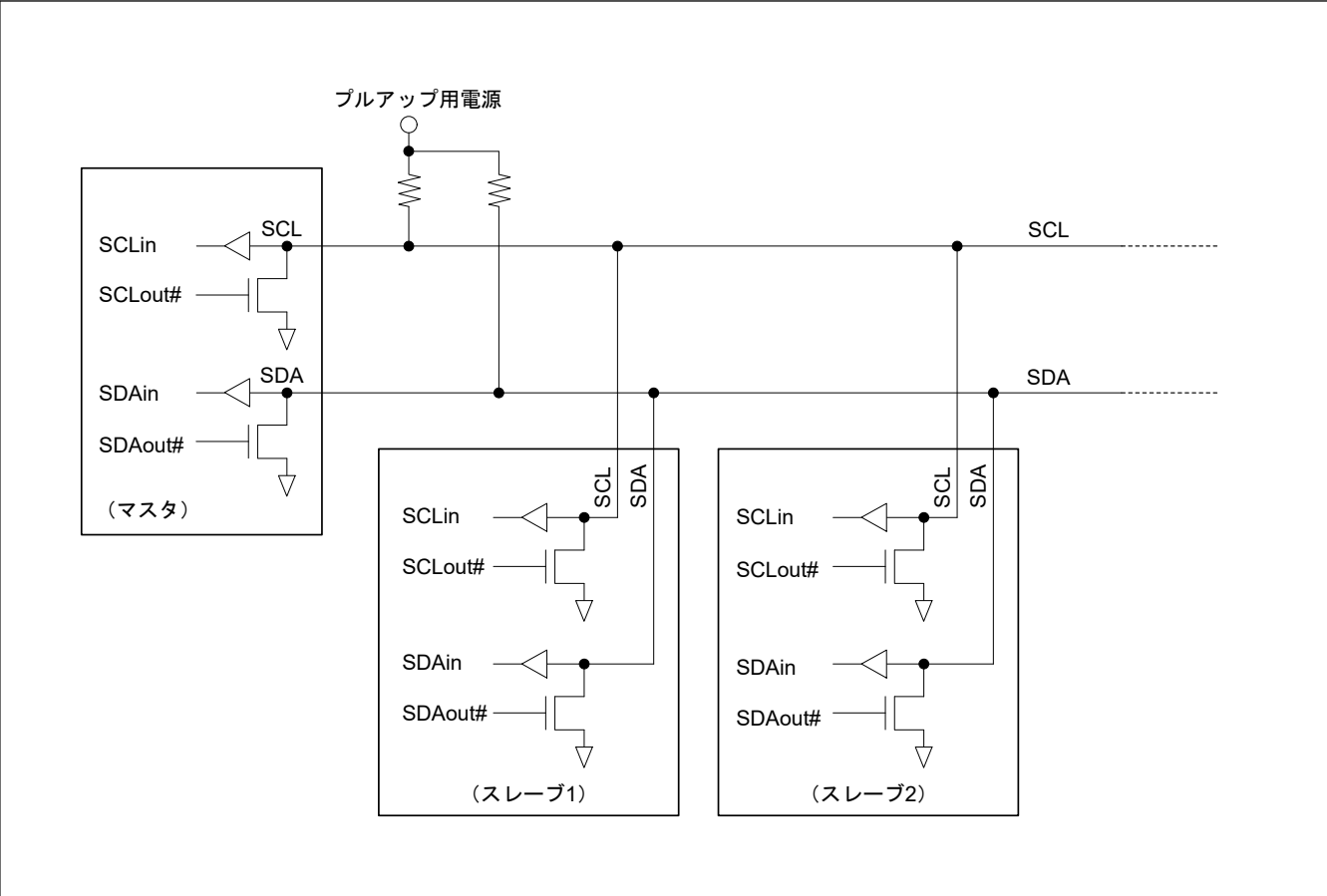
図 25.2 入出力端子の外部回路接続例 (I 2 C バス構成例)
