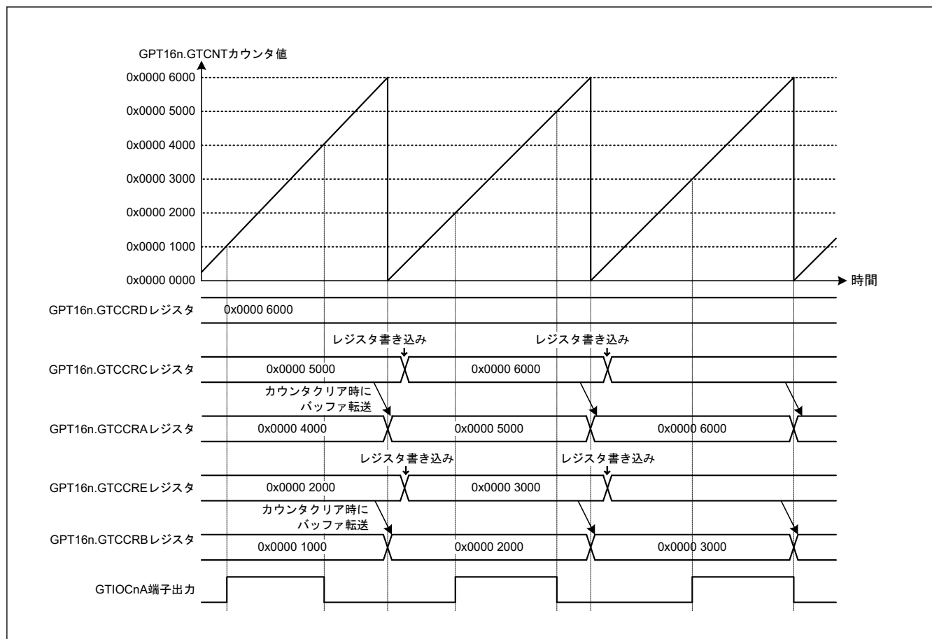
図 20.40 のこぎり波 PWM モード 2 の動作例 (GTCCRA レジスタコンペアマッチ時に Low 出力、GTCCRB レジスタコンペアマッチ時に High 出力、周期の終わりに Low 出力、シングルバッファ動作、GTCCRD レジスタコンペアマッチ時にクリア、GTIOR.OAEOCD ビット = 0) (n = 0~2)
