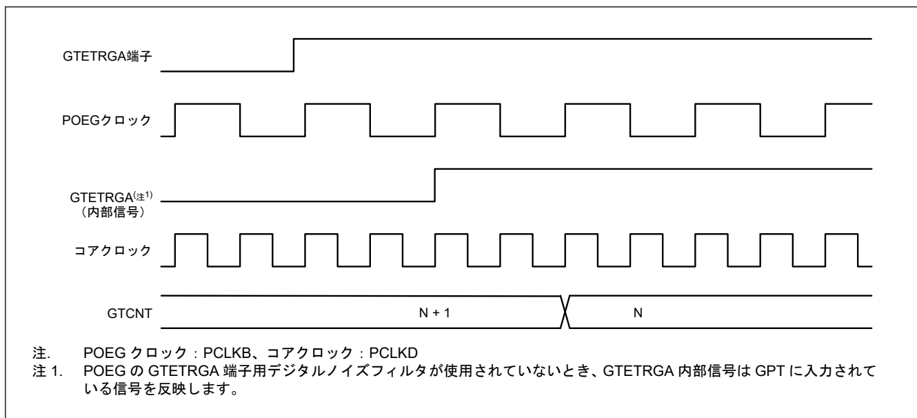
図 20.9 ハードウェア要因によるダウンカウント時のイベントカウント動作例
