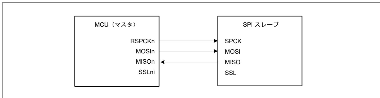
図 26.10 クロック同期式動作のマスタとスレーブの構成例 (MCU はマスタ)
