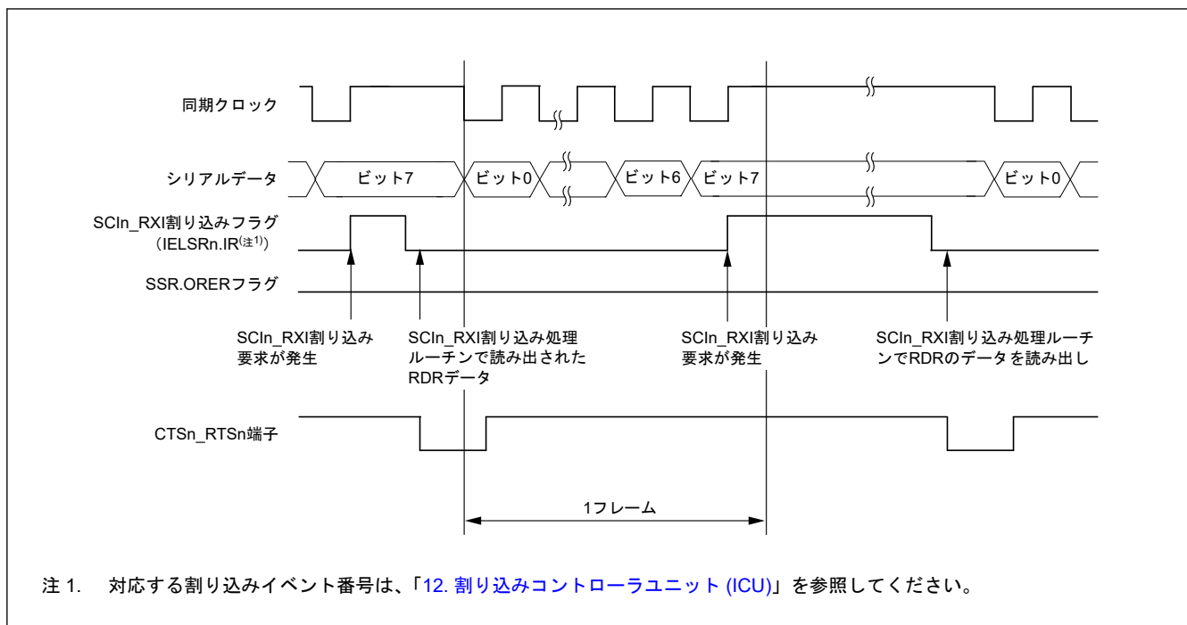
図 24.42 クロック同期式モードにおけるシリアル受信の動作例 (2) (RTS 機能を使用する場合)
