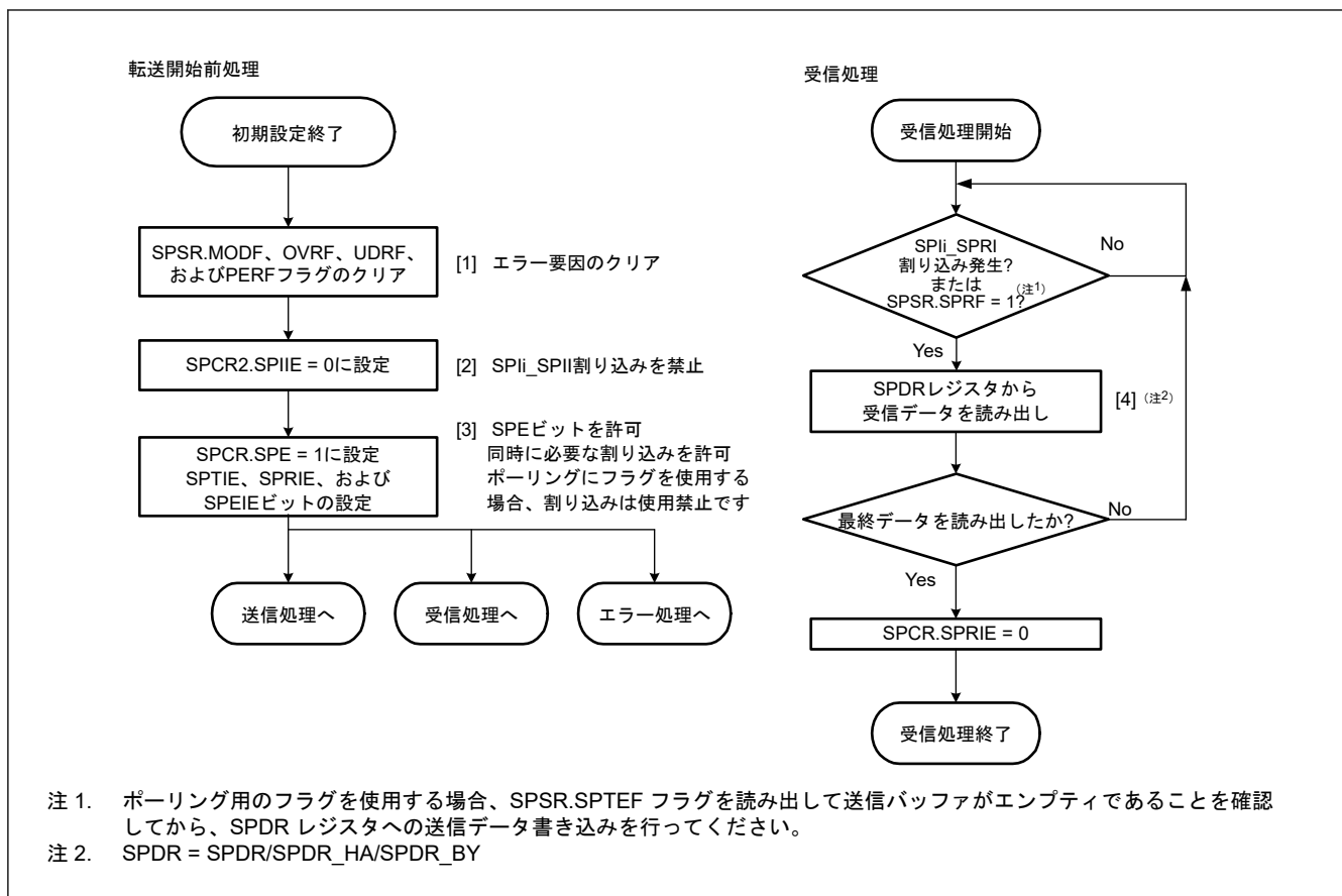
図 26.37 スレープモードでの受信フロー
