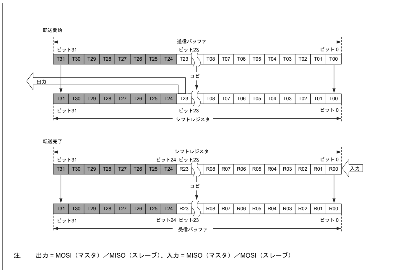
図 26.14 MSB ファースト転送 (24 ビットデータ/パリティ機能無効)
