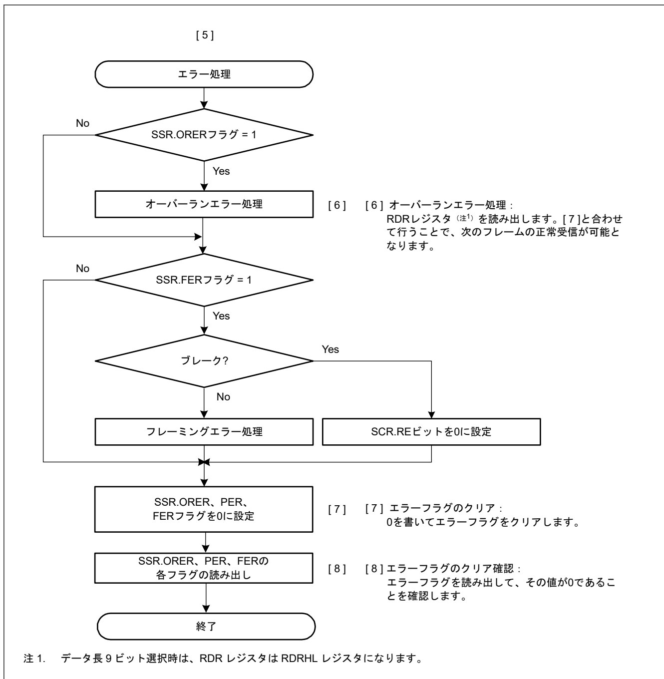
図 24.32 マルチプロセッサシリアル受信のフローチャート例（非 FIFO 選択時）(2)
