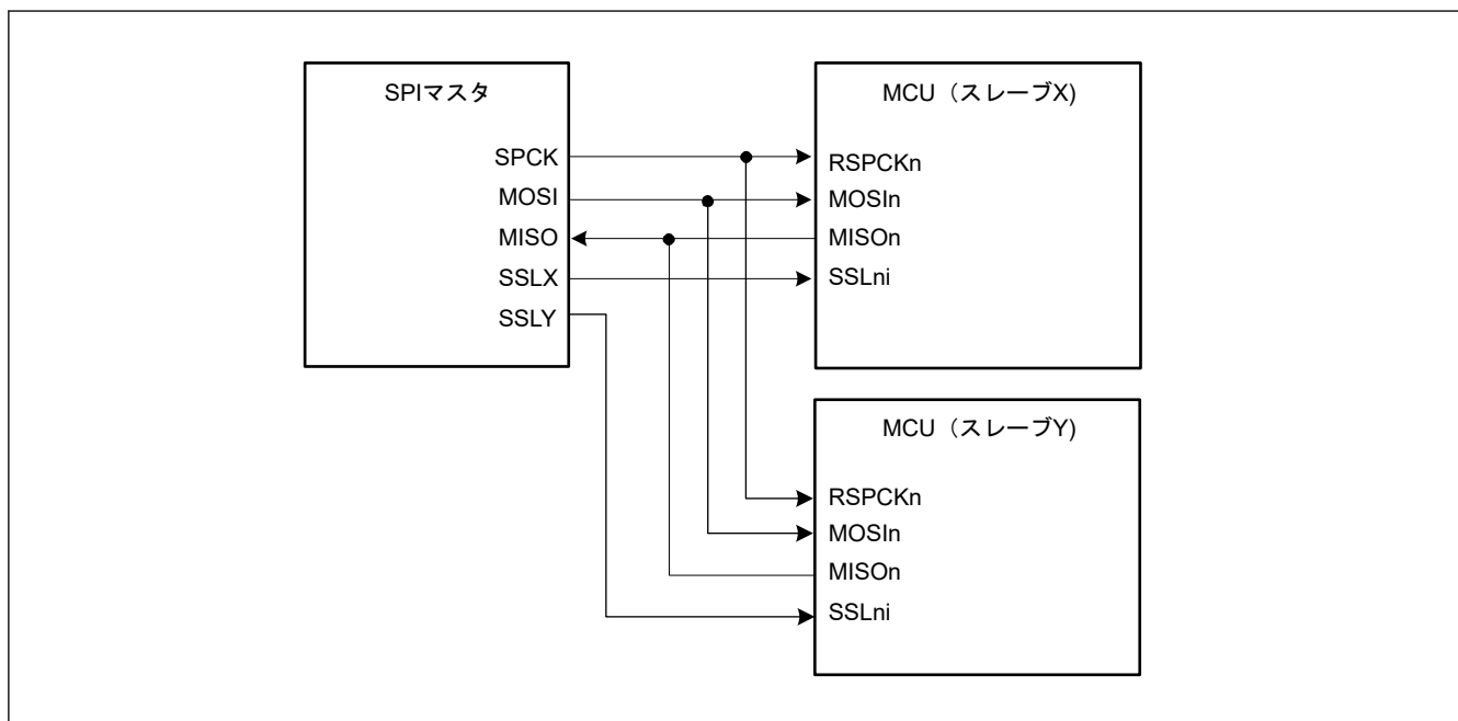
図 26.9 シングルマスタとマルチスレーブの構成例 (MCU はスレーブ)
