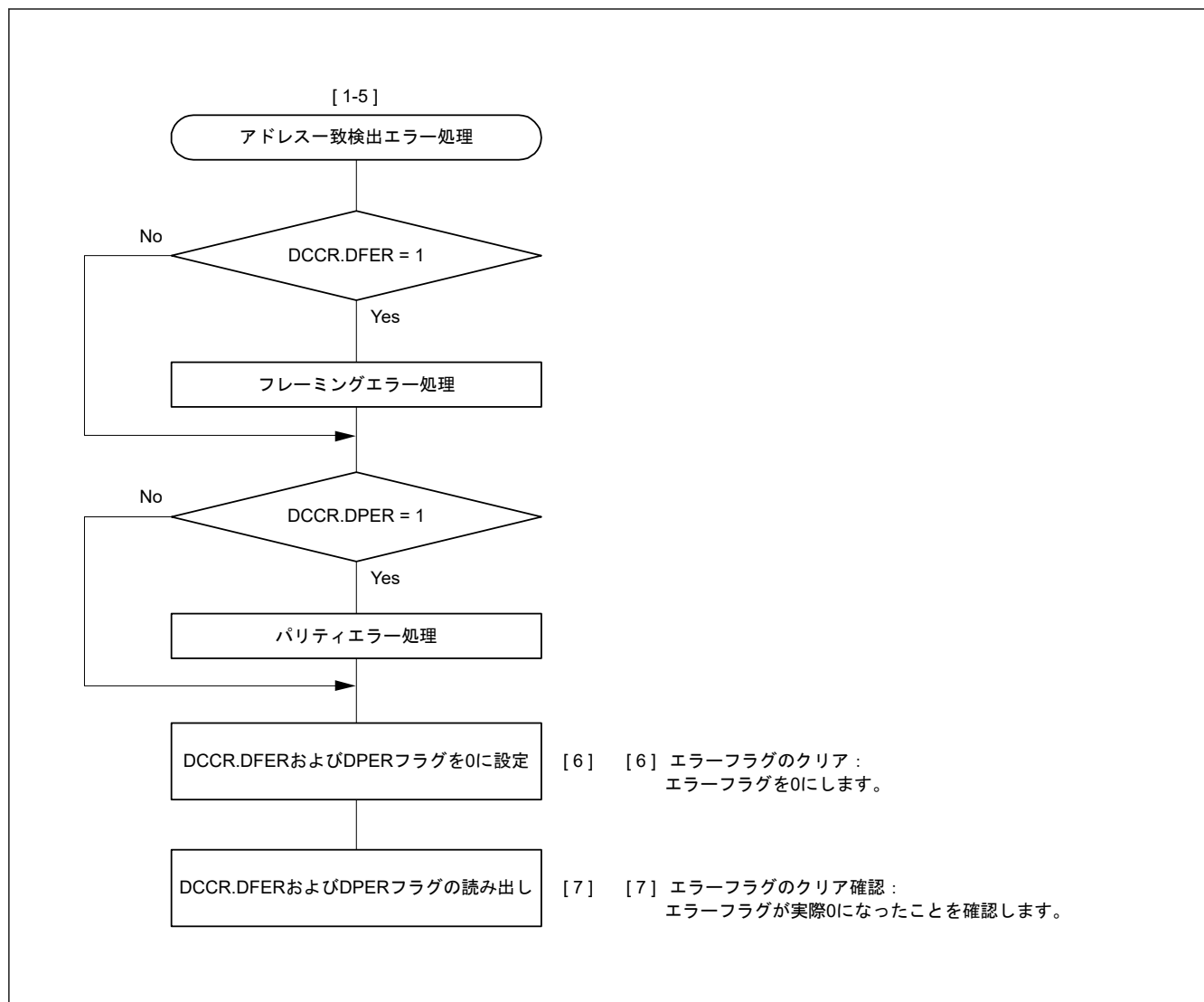
図 24.18 調歩同期式モードにおけるシリアル受信のフローチャート例（非 FIFO 選択、アドレス一致検出有効時） (2)
