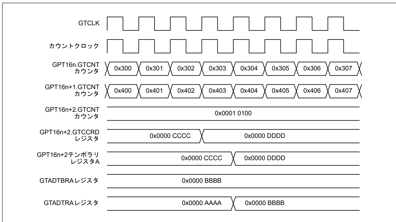
図 20.34 GTADTRA および GTADTRB レジスタのバッファ動作例 (相補 PWM モードでスレーブチャンネル 2 の GTCCRD レジスタが更新)
