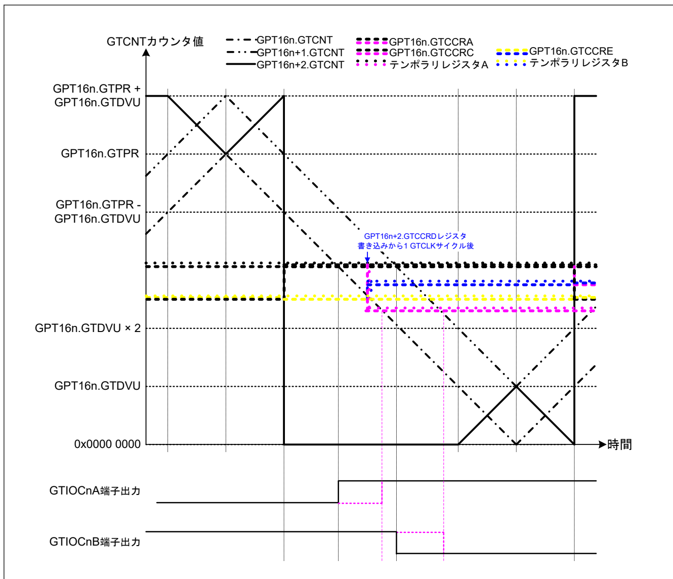
図 20.78 相補 PWM モード 4 のダブルバッファ動作例（ダウンカウント中間部分）（相補 PWM モード 4 ダブルバッファ動作、アップカウントの GTCCRA レジスタコンペアマッチ時：GTIOCN A 端子 = Low/GTIOCN B 端子 = High、ダウンカウントの GTCCRA レジスタコンペアマッチ時：GTIOCN A 端子 = High/GTIOCN B 端子 = Low、ダウンカウントデッドタイム時に値が GTCCRD レジスタに書き込まれた場合）（n = 0）
