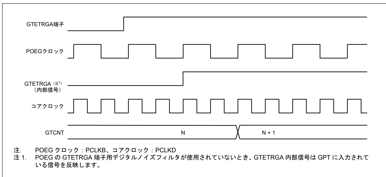
図 20.6 ハードウェア要因によるアップカウント時のイベントカウント動作例
