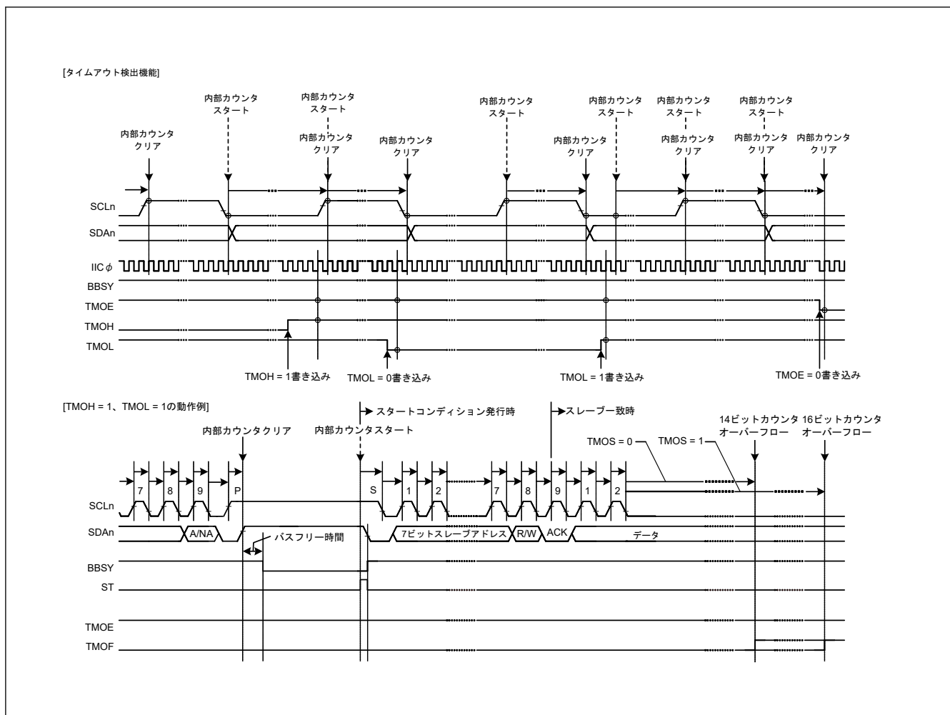
図 25.48 タイムアウト検出機能 (TMOE、TMOS、TMOH、TMOL ビットの使用)
