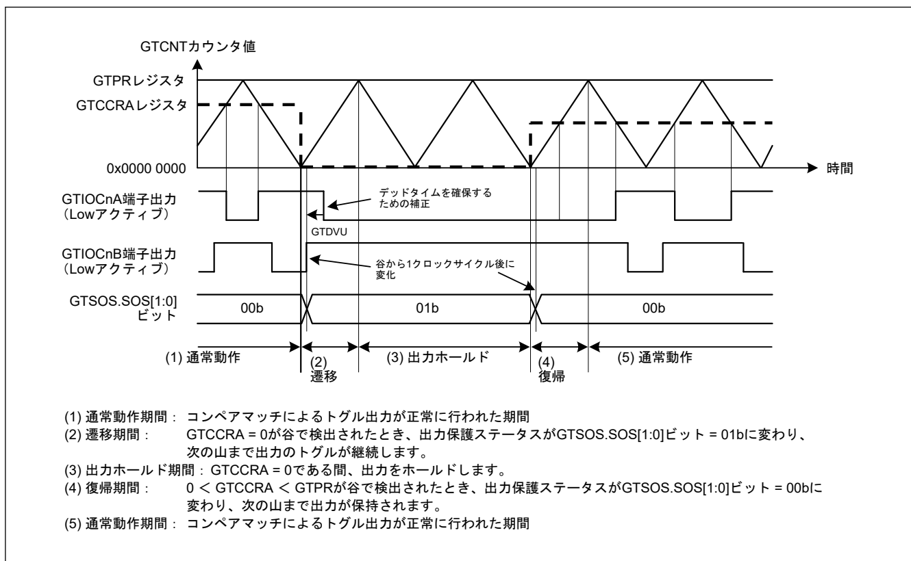
図 20.172 谷でのバッファ転送中に GTCCRA が 0x0000 0000 になったときの出力保護機能の動作例（谷でのバッファ転送中に 0 < GTCCRA < GTPR に復帰、アクティブレベル：Low）(n = 0 ~ 2)
