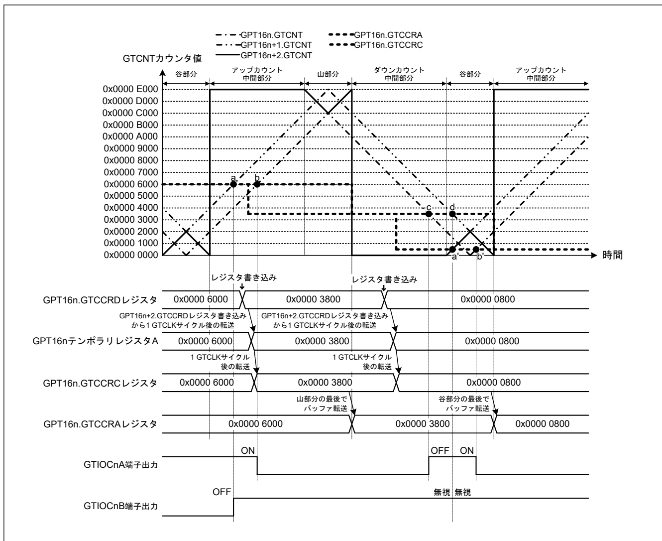
図 20.62 相補 PWM モードでのコンペアマッチ発生シーケンス動作例 (相補 PWM モード 3 シングルバッファ動作、アップカウントの GTCCRA レジスタコンペアマッチ時: GTIOCnA 端子 = Low/GTIOCnB 端子 = High、ダウンカウントの GTCCRA レジスタコンペアマッチ時: GTIOCnA 端子 = High/GTIOCnB 端子 = Low、デッドタイム値: 0x0000 2000、コンペアマッチ発生順序: c → (d, a') → b') (n = 0)
