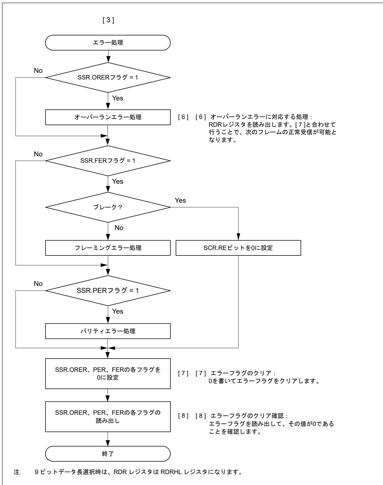
図 24.16 調歩同期式モードにおけるシリアル受信のフローチャート例（非 FIFO 選択、アドレス一致検出無効時） (2)
