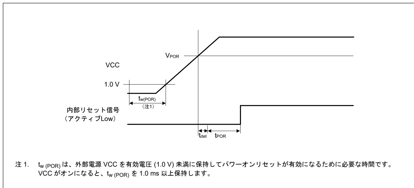
図 35.53 パワーオンリセットタイミング
