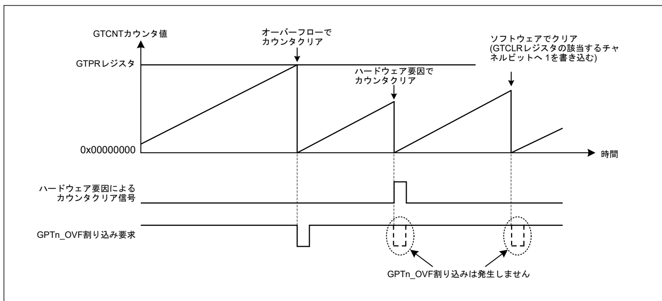
図 20.100 ハードウェア要因によるカウンタクリアと GPTn_OVF (n = 0~3) 割り込みの関係
