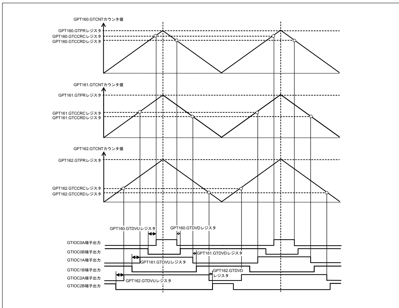
図 20.120 非対称三角波 3 相相補 PWM 出力例 (デッドタイム自動設定)
