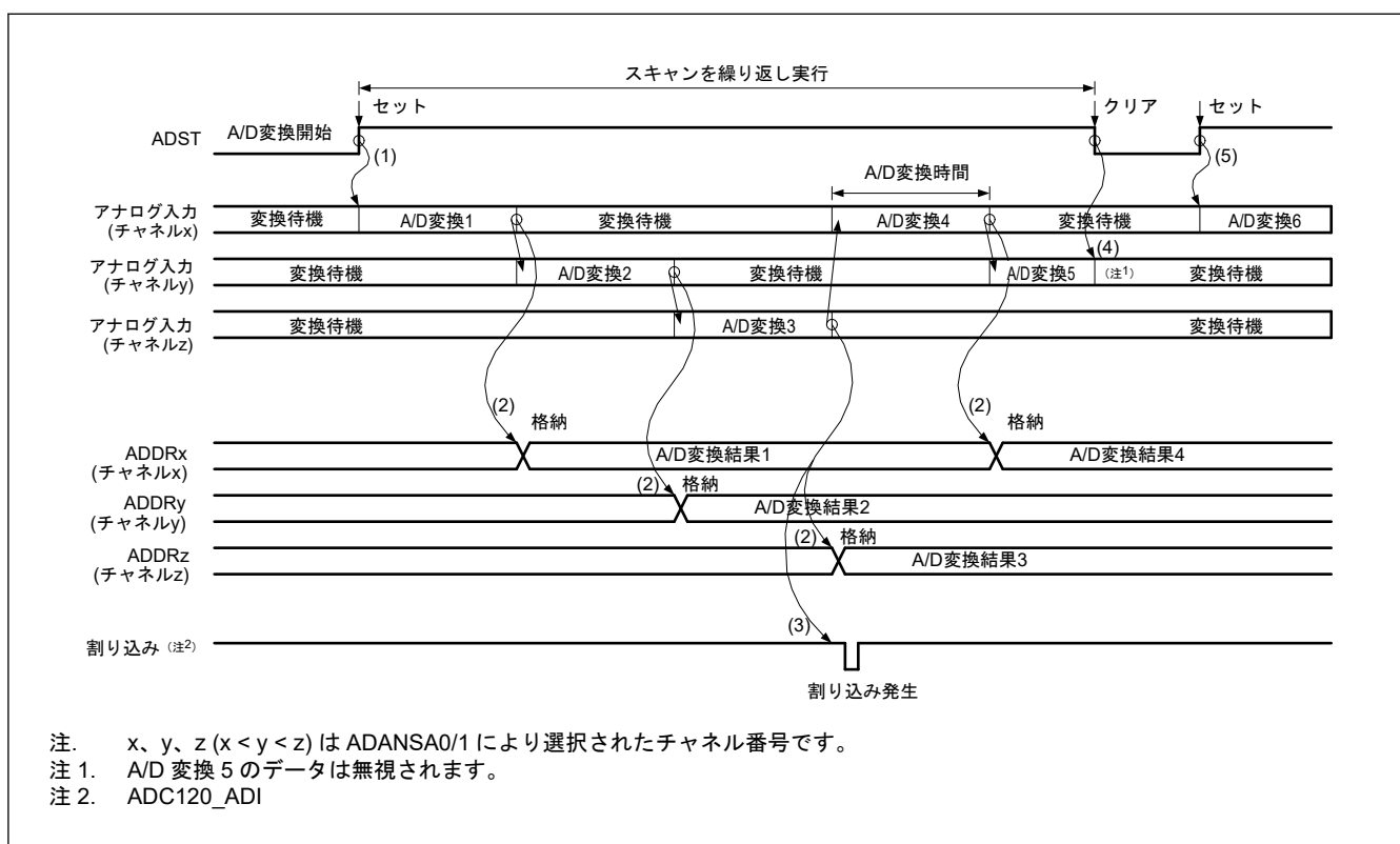
図 29.14 連続スキャンモードの基本動作例（アナログ入力（チャンネル x~z）選択）
