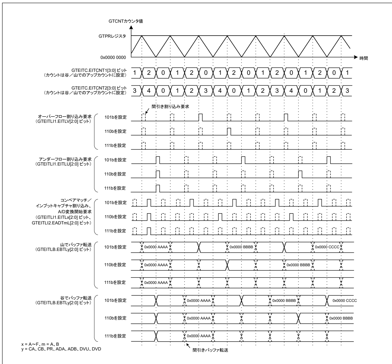
図 20.152 拡張割り込み間引き機能の動作例（三角波、山と谷の両方でカウント、拡張割り込み間引き 1 間引きカウント：2、山と谷の両方でカウント、拡張割り込み間引き 2 間引きカウント：4、拡張割り込み間引きカウンタ 2 の初期値：0、GTEITC.EITCNTk ビット (k = 1, 2) が GTEITC.EIVTTk ビット以外の期間で間引き)
