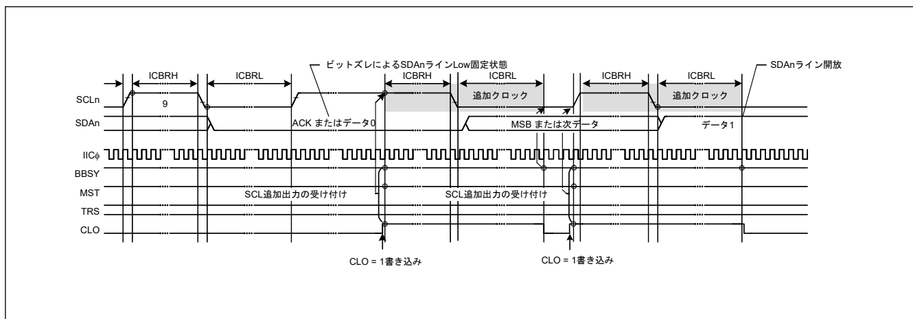
図 25.49 SCL クロック追加出力機能 (CLO ビット)
