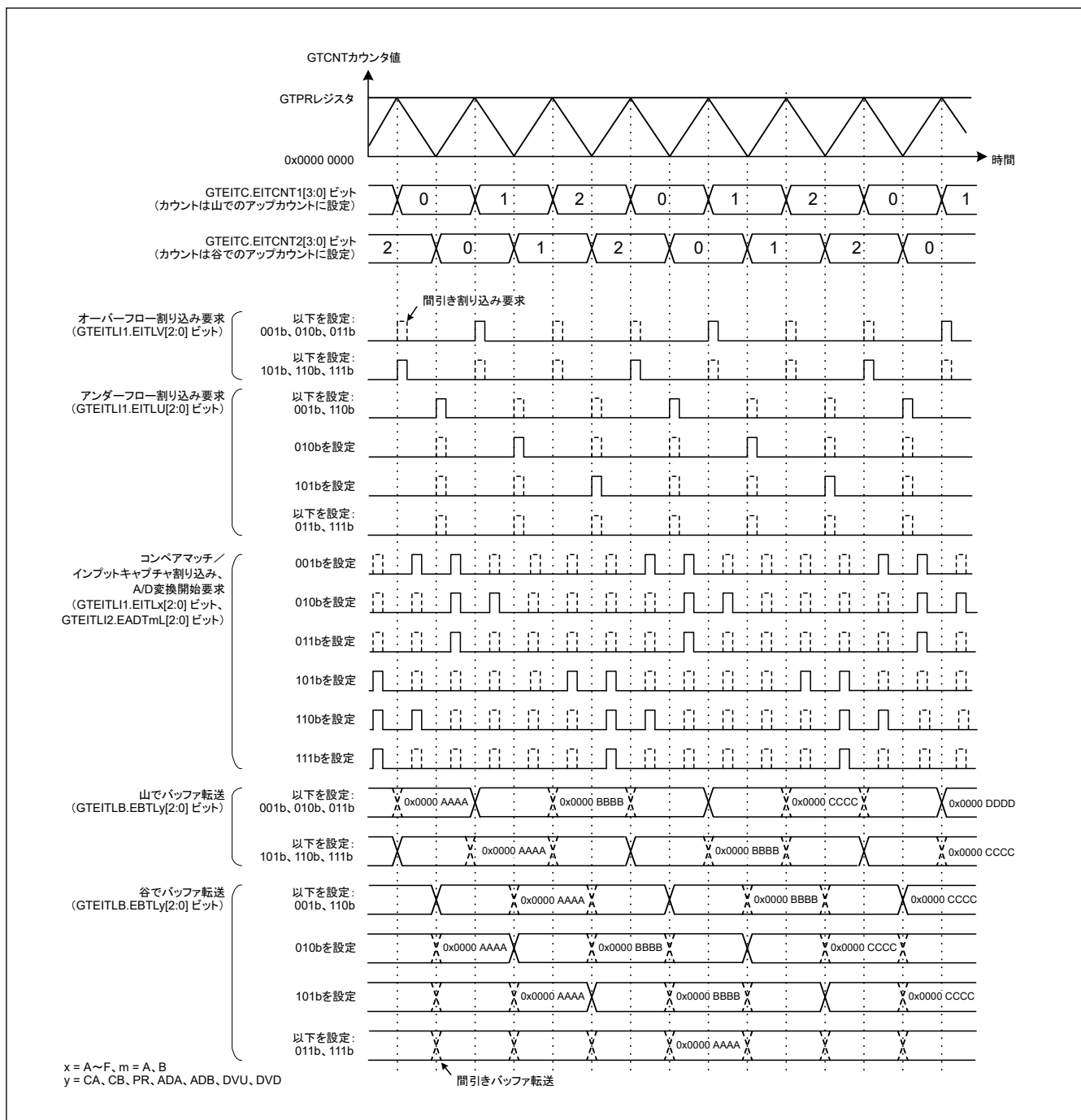
図 20.147 拡張割り込み間引き機能の例 (三角波、山でカウント、拡張割り込み間引き 1 間引きカウント : 2、谷でカウント、拡張割り込み間引き 2 間引きカウント : 2、拡張割り込み間引きカウンタ 2 の初期値 : 0)
