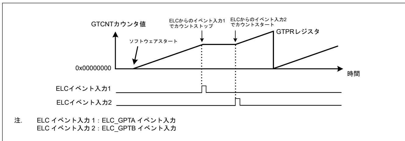
図 20.93 ハードウェア要因によるカウントストップ動作例（ソフトウェアによるスタート、ELC_GPTA 入力でのストップ、ELC_GPTB 入力での再スタートの場合）
