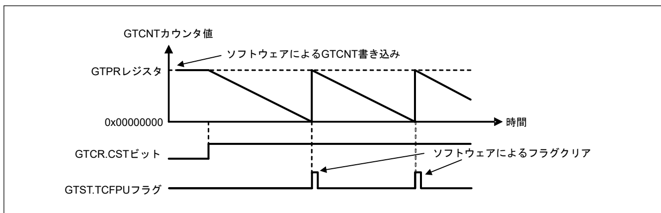
図 20.5 カウントクロックによるダウンカウント時の周期カウント動作例
