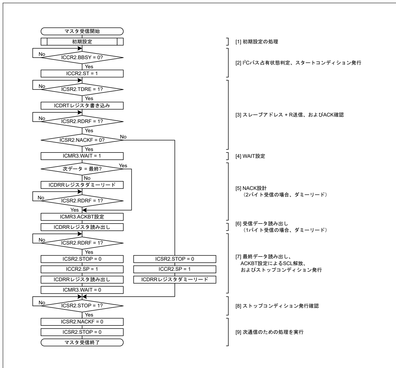
図 25.10 マスタ受信の例 (7ビットアドレスフォーマットで1または2バイト受信の場合)
