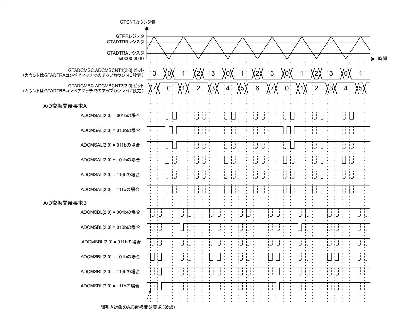
図 20.158 A/D 変換開始要求コンペアマッチ間引き機能の動作例 (三角波、A/D 変換開始要求コンペアマッチ間引き 1 間引きカウント : 3 カウント GTADTRA コンペアマッチ、A/D 変換開始要求コンペアマッチ間引き 2 間引きカウント : 7 カウント GTADTRB コンペアマッチ)
