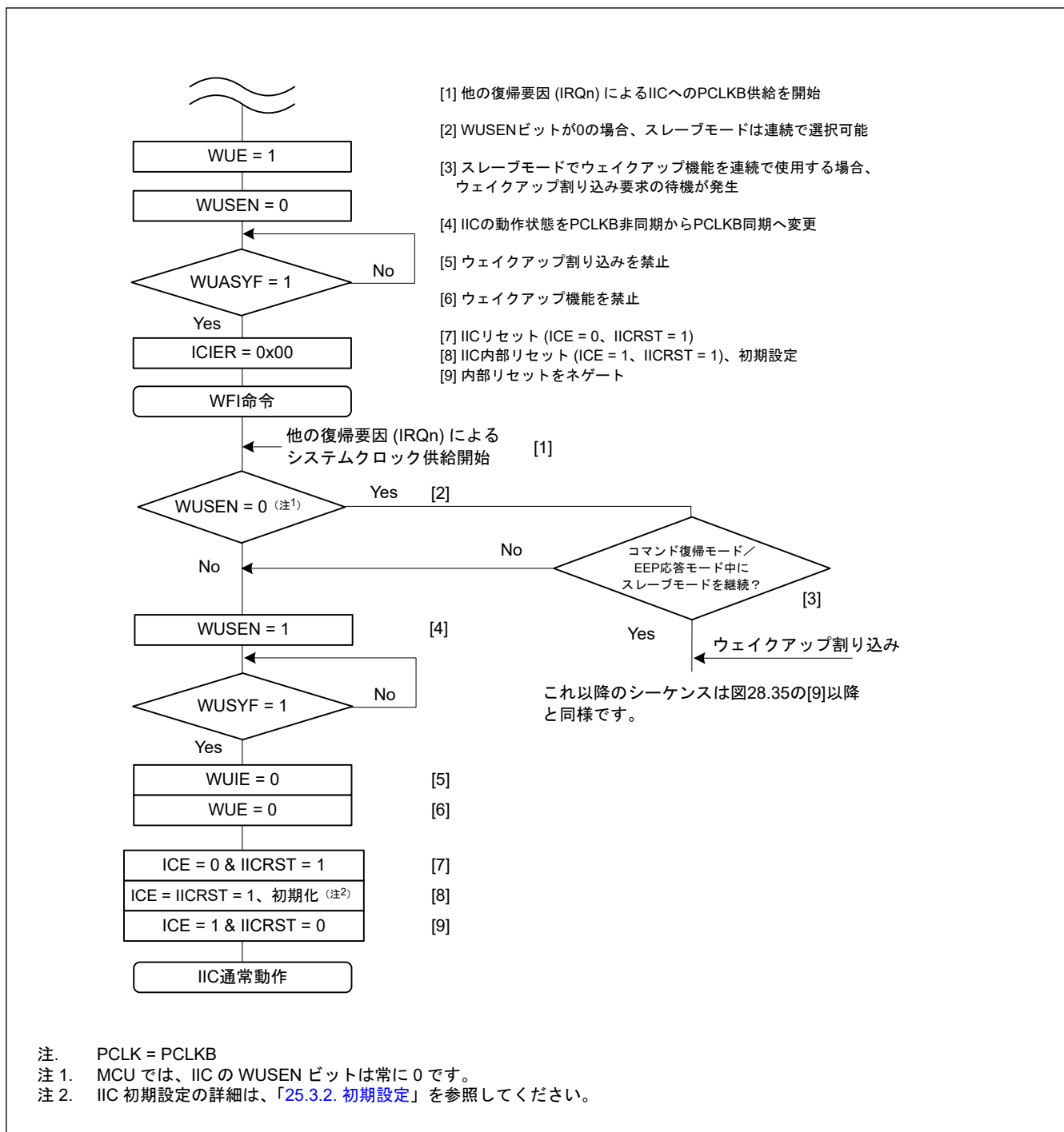
図 25.36 コマンドリカバリモードとEEP 応答モードの動作例 (IIC ウェイクアップ割り込み以外の割り込み (たとえば IRQn) によるウェイクアップの場合)
