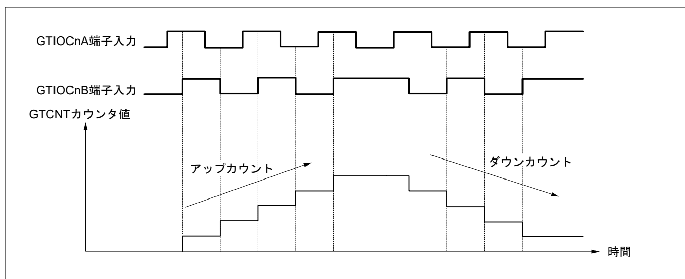
図 20.130 位相計数モード 4 の動作例
