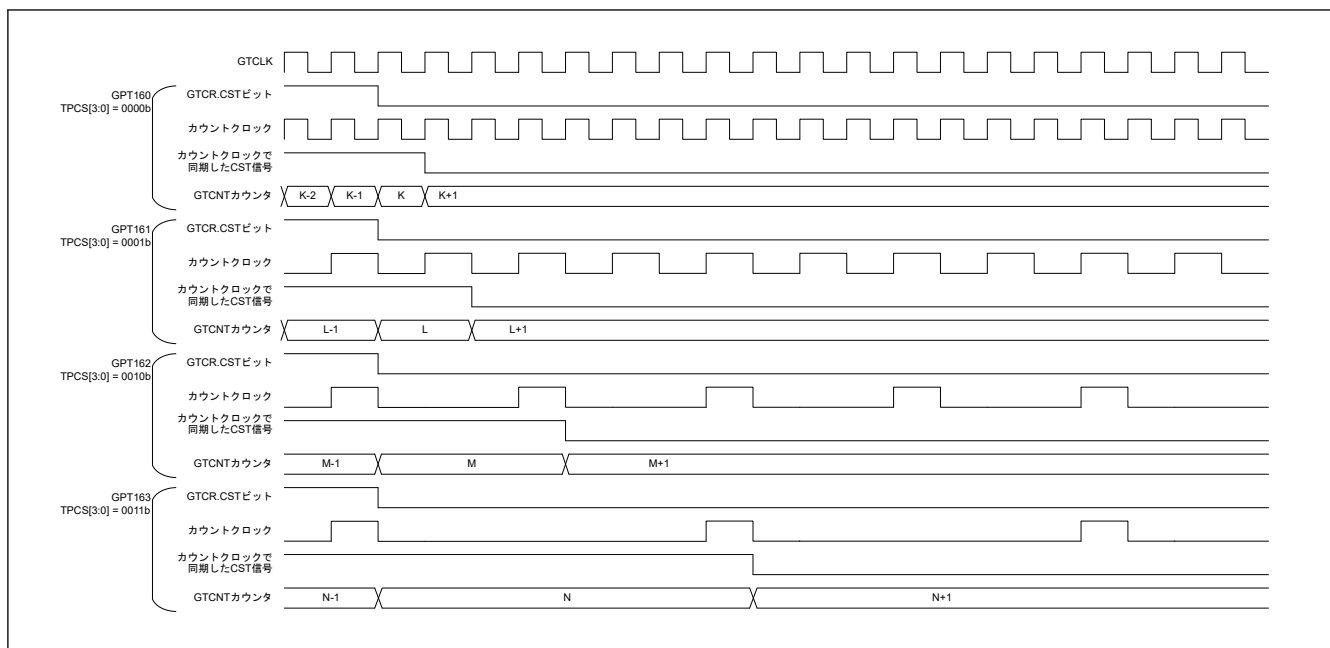
図 20.110 ソフトウェアによる同時ストップの動作例 (異なるカウント周期)
