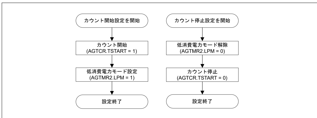
図 21.2 LPM ビットに書き込む方法のフローチャート
