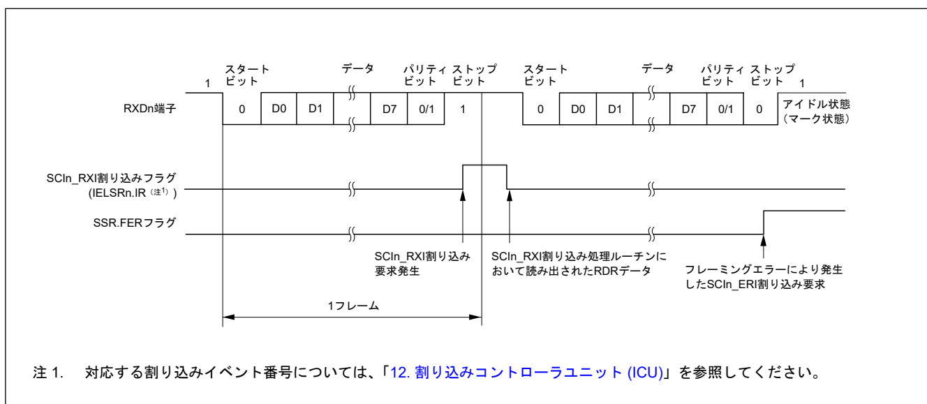
図 24.13 調歩同期式モードにおけるシリアル受信の動作例 (1) (RTS 機能を使用しない場合) (8 ビットデータ/パリティあり/1 ストップビットの場合)
