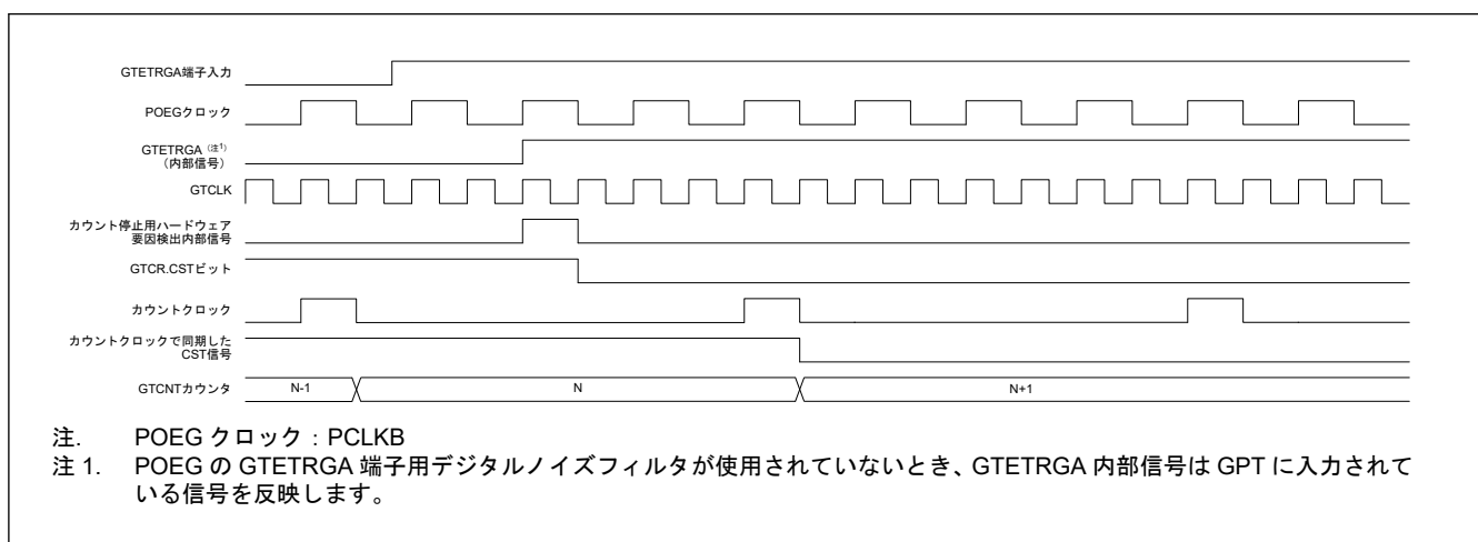
図 20.95 GTETRGA 端子の入力の立ち上がりエッジに対応するカウントストップ動作のタイミング例
