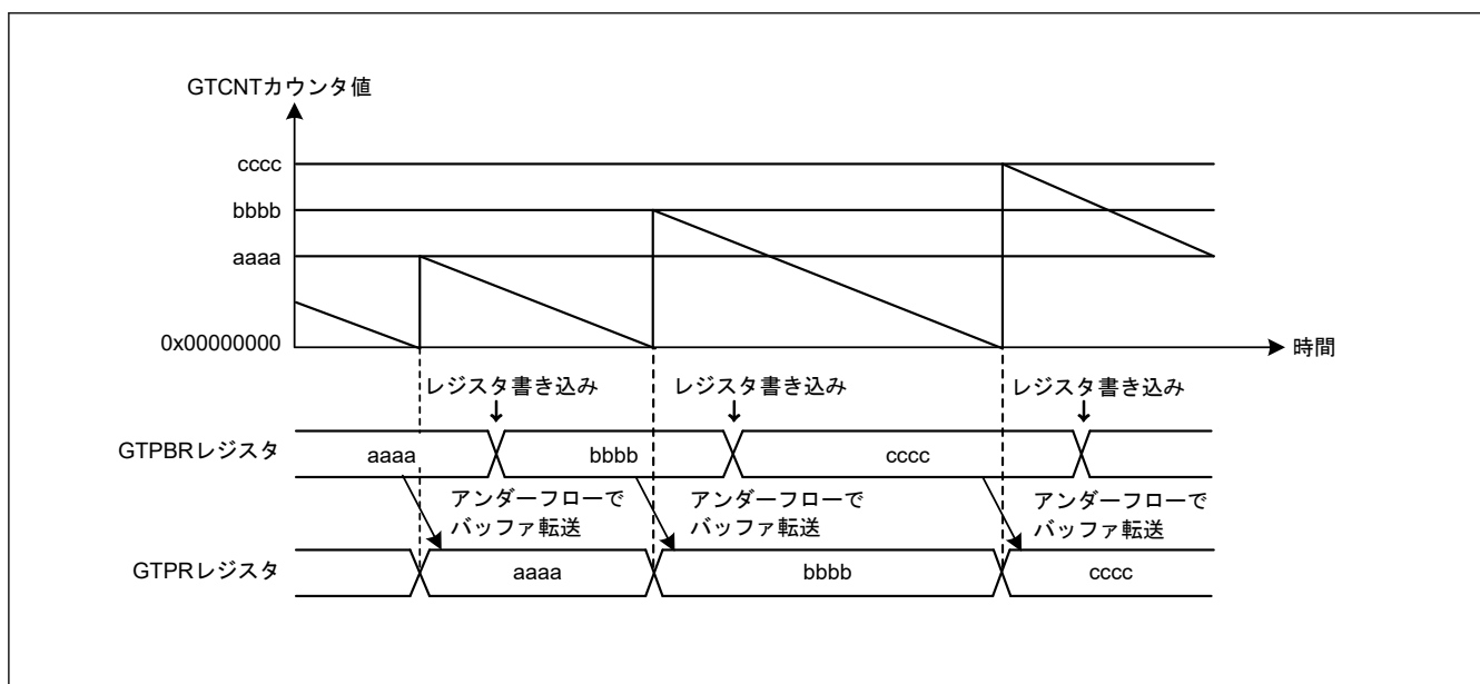
図 20.19 GTPR レジスタのバッファ動作例 (のこぎり波でダウンカウントの場合)
