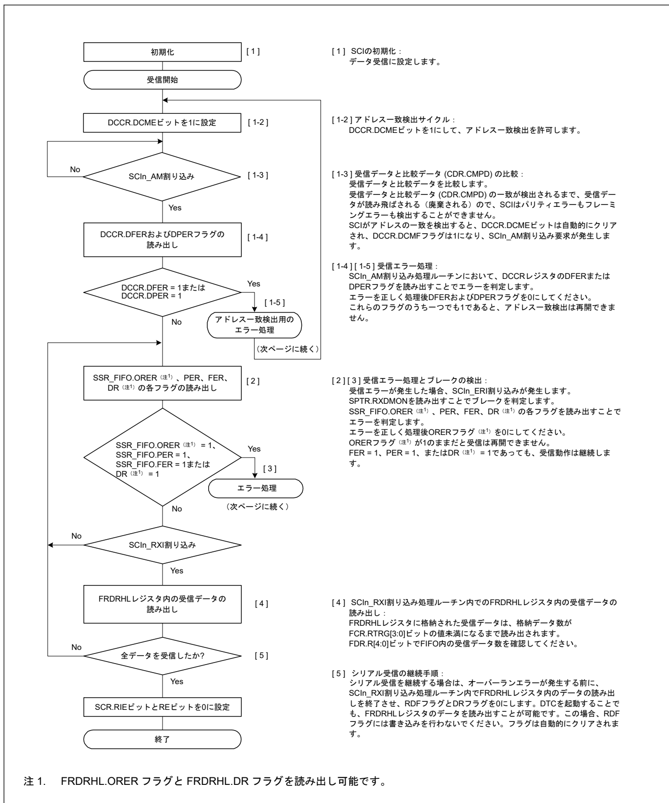
図 24.23 調歩同期式モードにおけるシリアル受信のフローチャート例 (FIFO 選択、アドレス一致検出有効時) (1)
