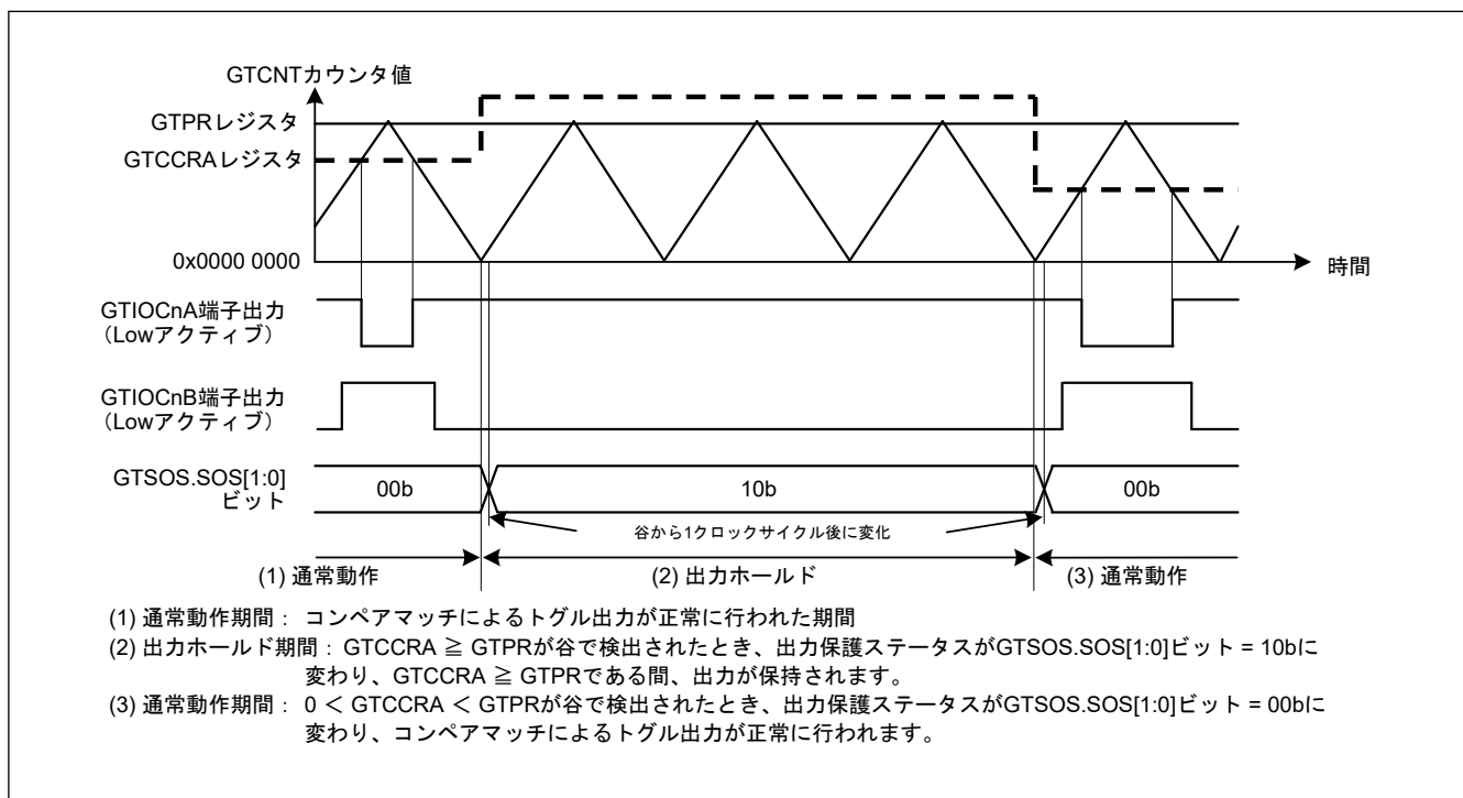
図 20.176 谷でのバッファ転送中に GTCCRA \geq GTPR となったときの出力保護機能の動作例（谷でのバッファ転送中に 0 < \text{GTCCRA} < \text{GTPR} に復帰、アクティブレベル：Low）（ n = 0 \sim 2 ）
