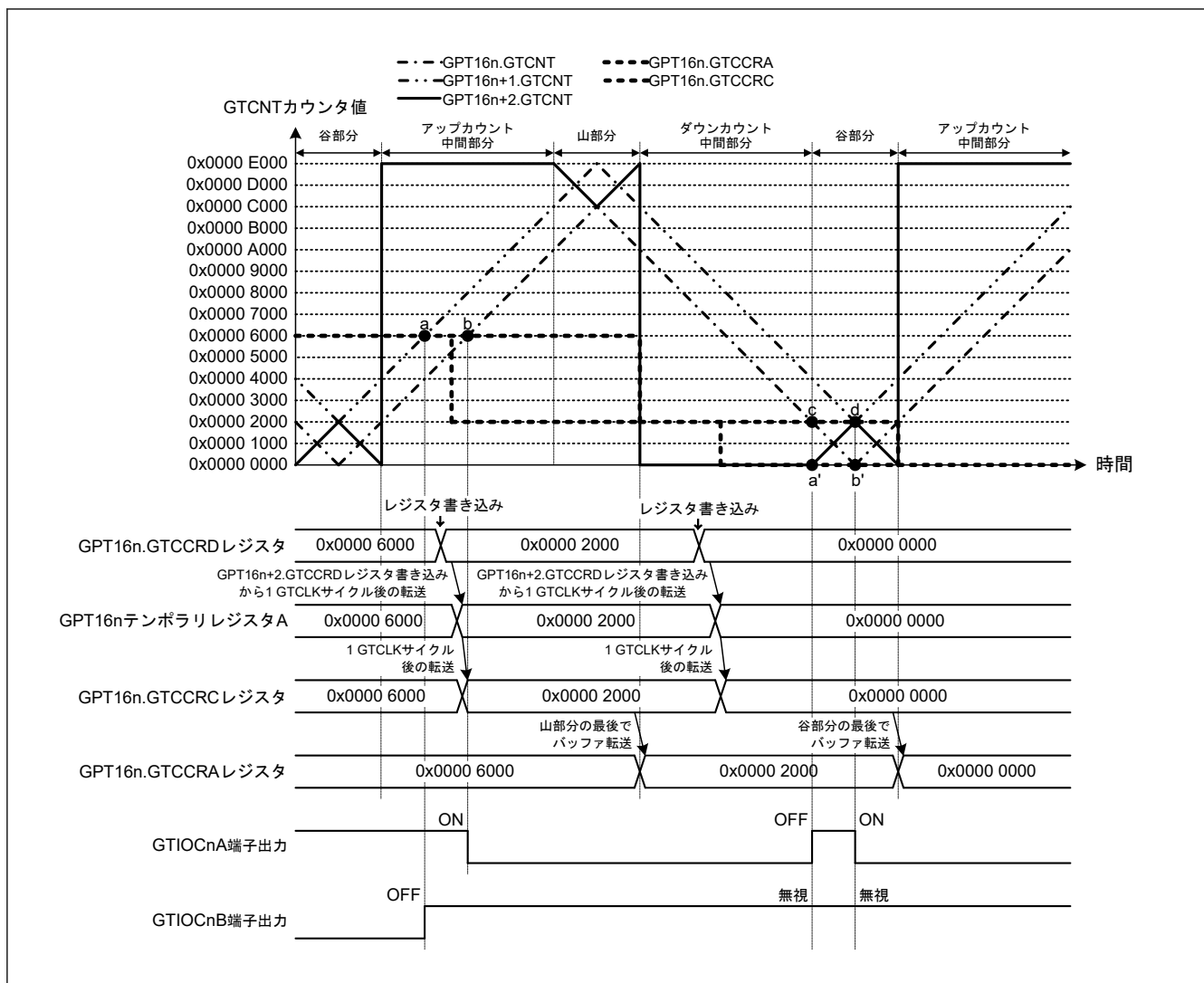
図 20.64 相補 PWM モードでのコンペアマッチ発生シーケンス動作例 (相補 PWM モード 3 シングルバッファ動作、アップカウントの GTCCRA レジスタコンペアマッチ時: GTIOcNA 端子 = Low/GTIOcNB 端子 = High、ダウンカウントの GTCCRA レジスタコンペアマッチ時: GTIOcNA 端子 = High/GTIOcNB 端子 = Low、デッドタイム値: 0x0000 2000、コンペアマッチ発生順序: (c, a') → (d, b')) (n = 0)
