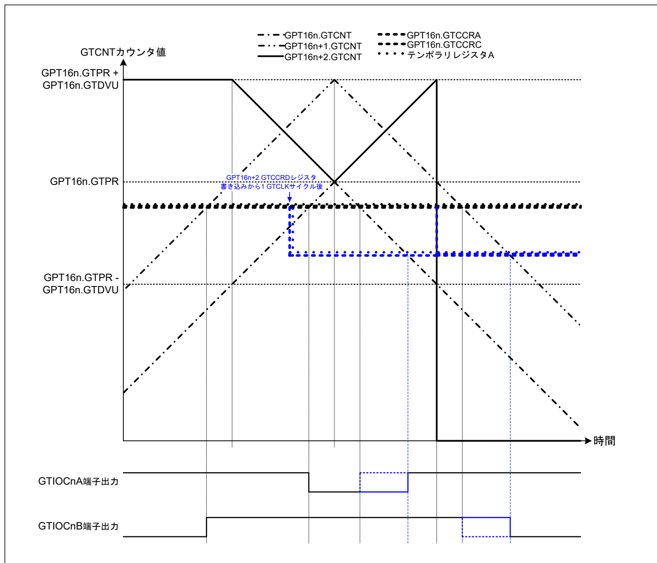
図 20.71 相補 PWM モード 4 のシングルバッファ動作例（アップカウント山部分）（相補 PWM モード 4 シングルバッファ動作、アップカウントの GTCCRA レジスタコンペアマッチ時：GTIOCnA 端子 = Low / GTIOCnB 端子 = High、ダウンカウントの GTCCRA レジスタコンペアマッチ時：GTIOCnA 端子 = High / GTIOCnB 端子 = Low、アップカウントデッドタイム時に値が GTCCRD レジスタに書き込まれた場合）（n = 0）
