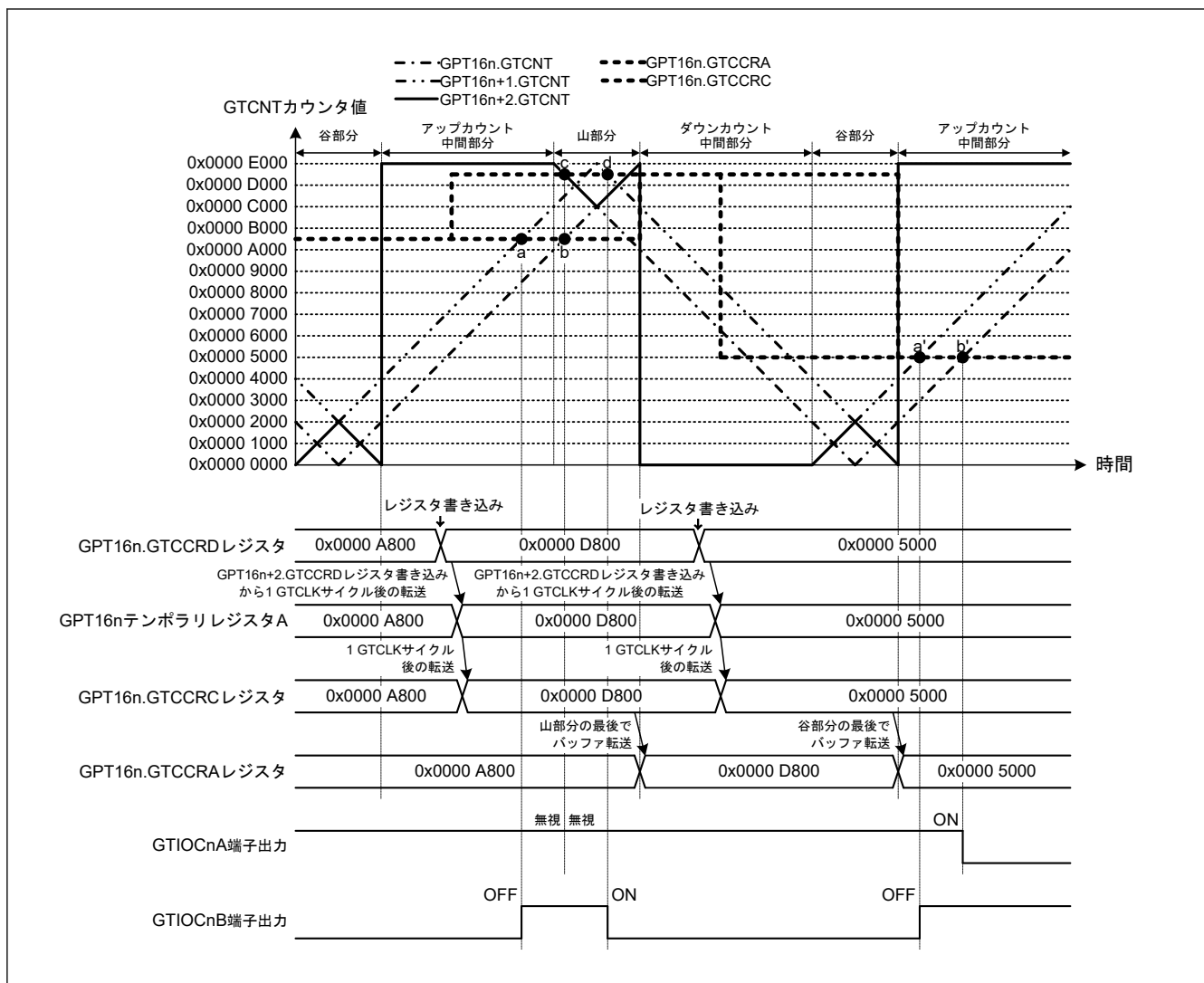
図 20.56 相補 PWM モードでのコンペアマッチ発生シーケンス動作例 (相補 PWM モード 3 シングルバッファ動作、アップカウントの GTCCRA レジスタコンペアマッチ時: GTIOcNA 端子 = Low/GTIOcNB 端子 = High、ダウンカウントの GTCCRA レジスタコンペアマッチ時: GTIOcNA 端子 = High/GTIOcNB 端子 = Low、デッドタイム値: 0x0000 2000、コンペアマッチ発生順序: a → (b, c) → d) (n = 0)
