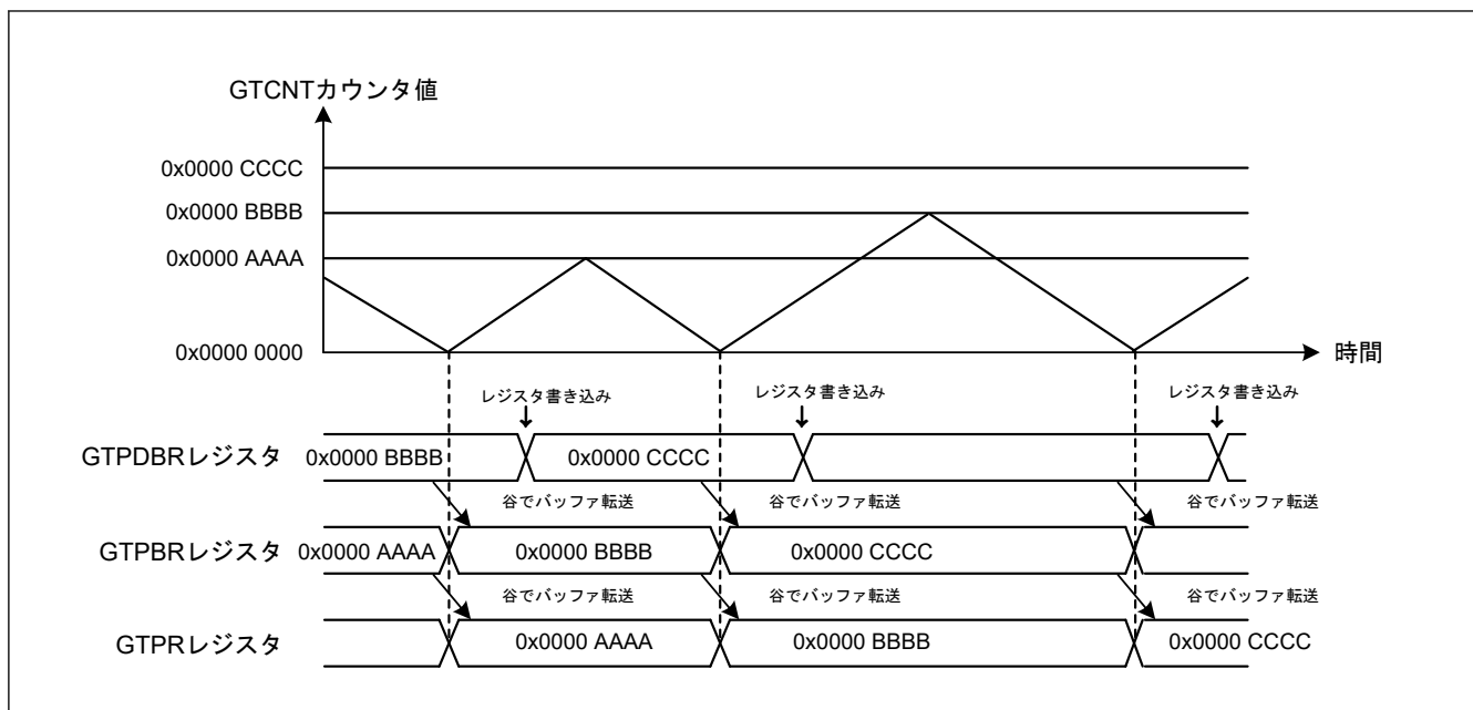
図 20.20 GTPR レジスタのダブルバッファ動作例 (三角波の場合)
