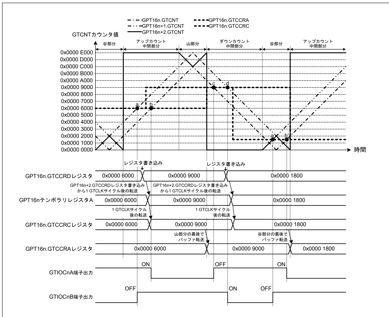
図 20.61 相補 PWM モードでのコンペアマッチ発生シーケンス動作例 (相補 PWM モード 3 シングルバッファ動作、アップカウントの GTCCRA レジスタコンペアマッチ時: GTIOcNA 端子 = Low/GTIOcNB 端子 = High、ダウンカウントの GTCCRA レジスタコンペアマッチ時: GTIOcNA 端子 = High/GTIOcNB 端子 = Low、デッドタイム値: 0x0000 2000、コンペアマッチ発生順序: c → d → a' → b') (n = 0)
