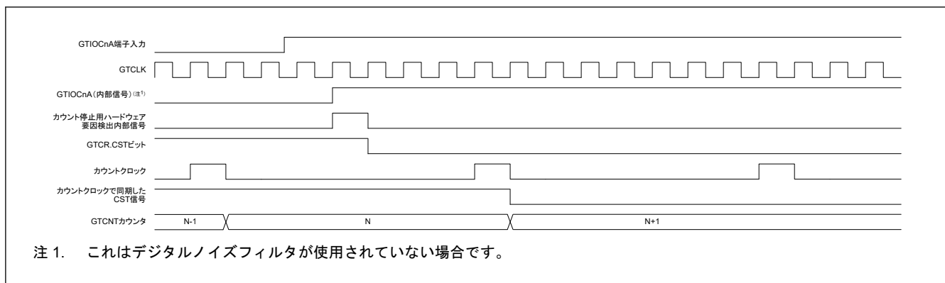
図 20.96 GTIOcNA 端子の入力の立ち上がりエッジに対応するカウントストップ動作のタイミング例
