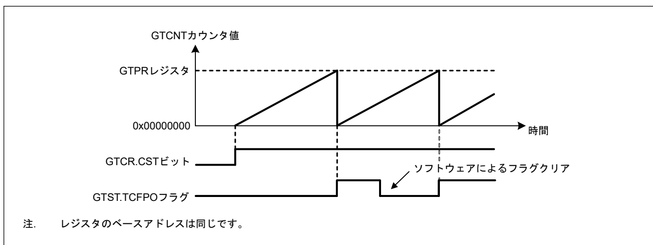
図 20.4 カウントクロックによるアップカウント時の周期カウント動作例
