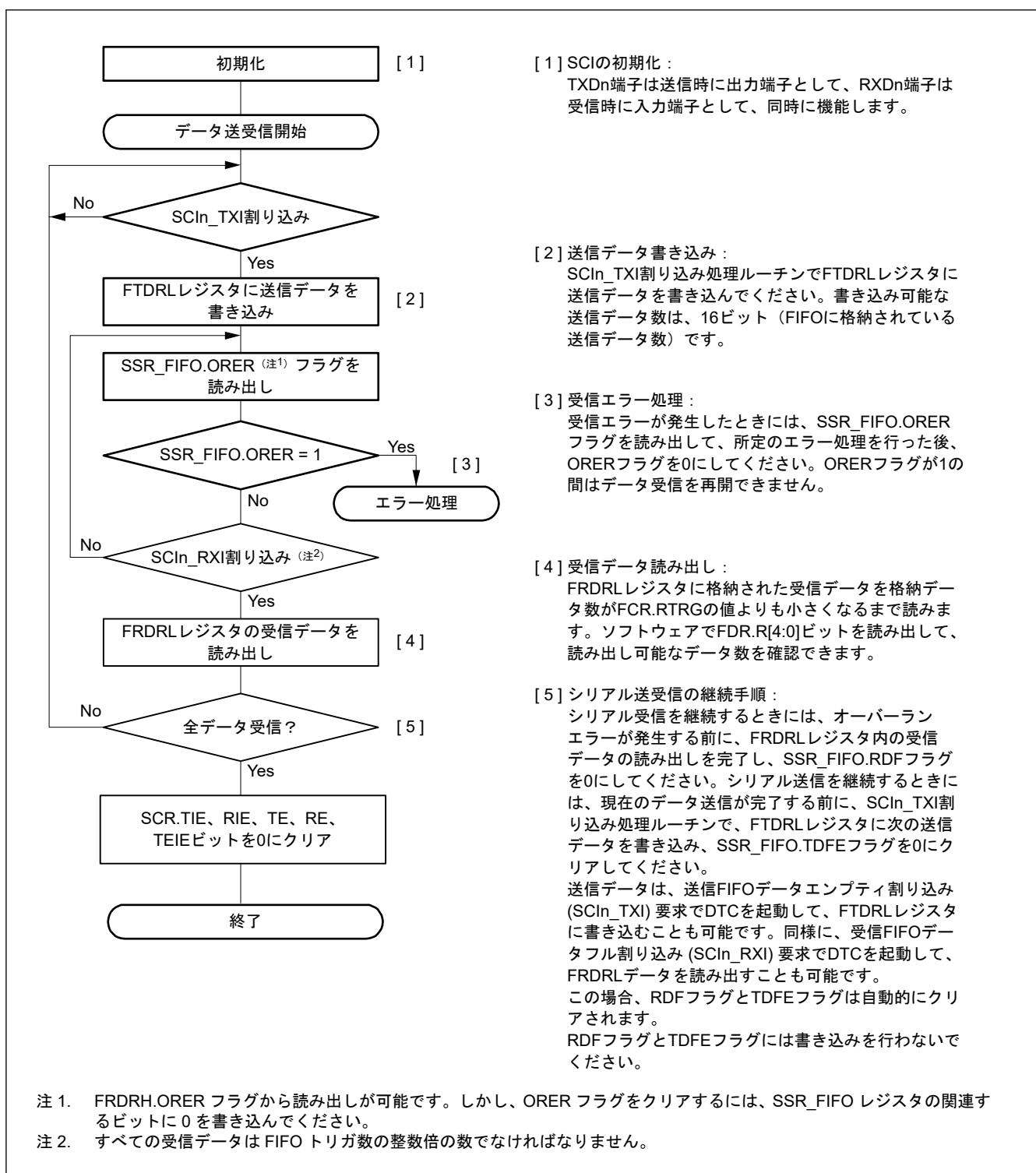
図 24.46 クロック同期式モードにおけるシリアル同時送受信動作のフローチャート例 (FIFO 選択時)
