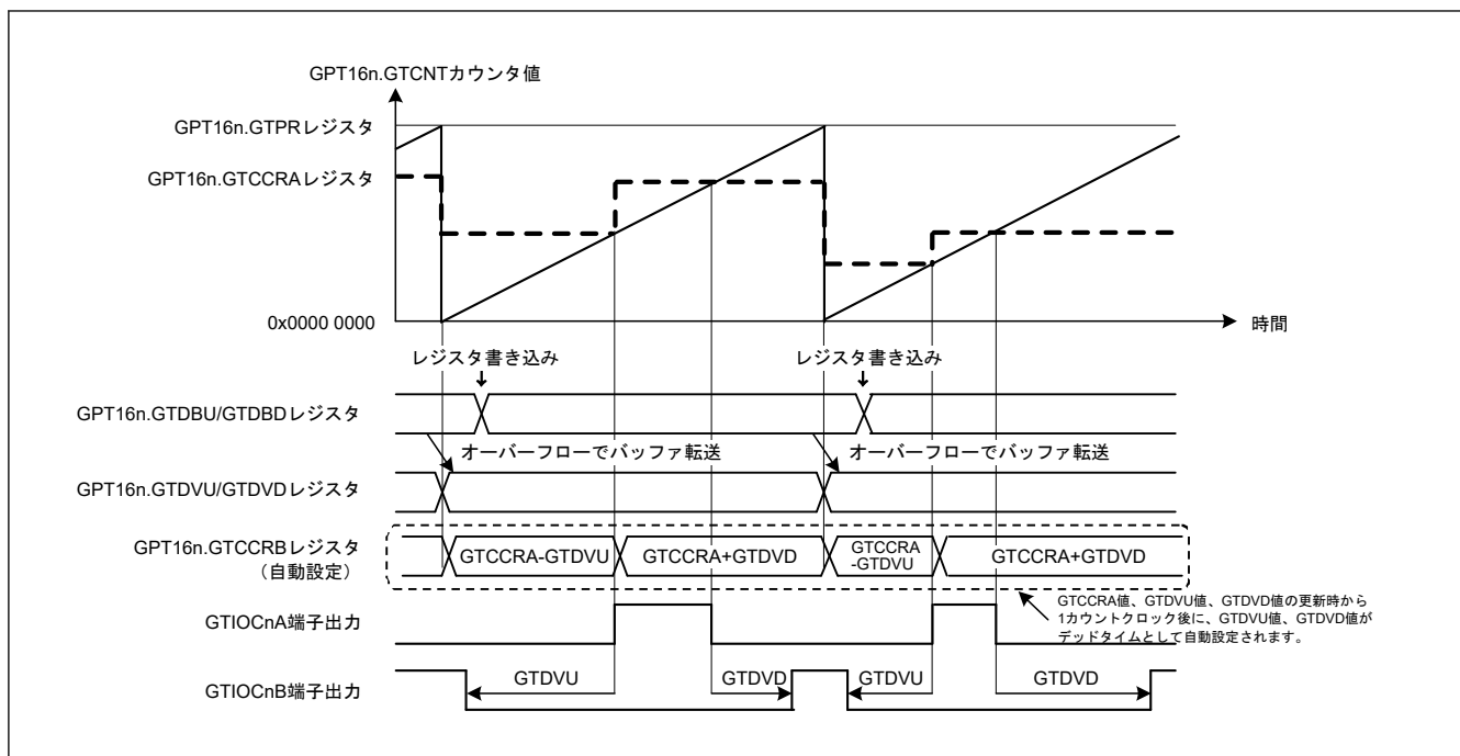
図 20.79 デッドタイム自動設定機能の動作例 (のこぎり波ワンショットパルスモード、アップカウント、GTDVU と GTDDVD はバッファ動作に設定、GPT160～GPT162 でアクティブ High の場合)
