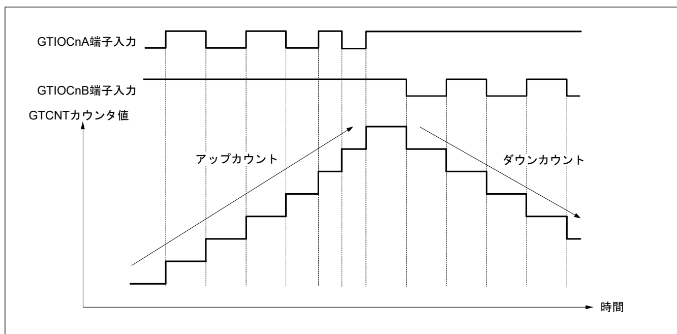
図 20.129 位相計数モード3の動作例 (C)
