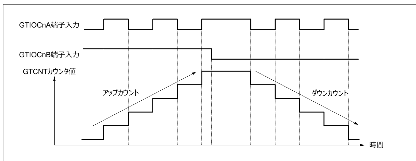
図 20.126 位相計数モード2の動作例 (C)
