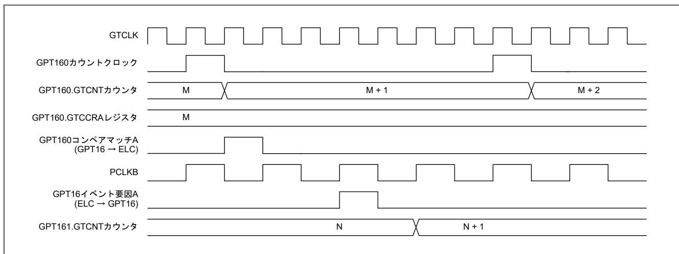
図 20.8 イベントカウンタ動作例 (ELC_GPTA からのイベント信号入力数のアップカウント時)
