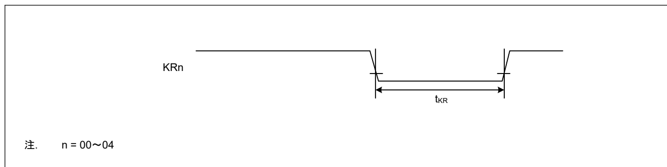
図 35.30 キー割り込み入力タイミング
