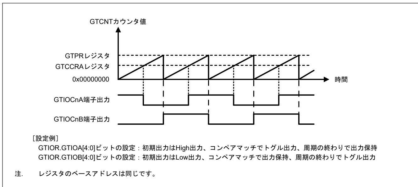
図 20.12 トグル出力動作例 (2)
