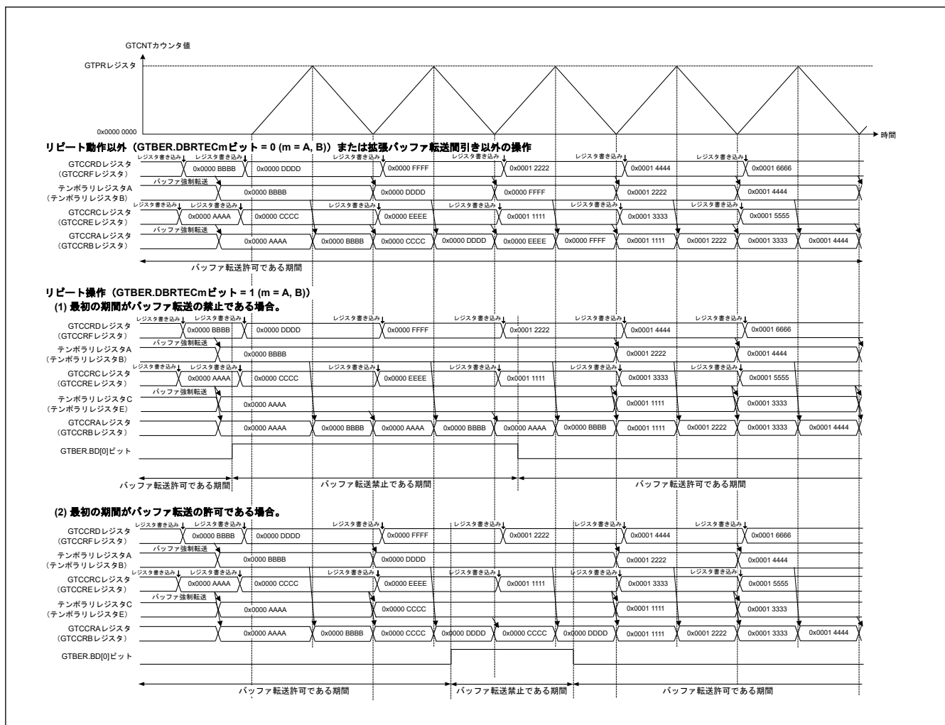
図 20.169 GTCCR バッファ転送が禁止されているときのリポートダブルバッファ動作例 (三角波 PWM モード 3、GTBER.BD[0]ビットを更新)
