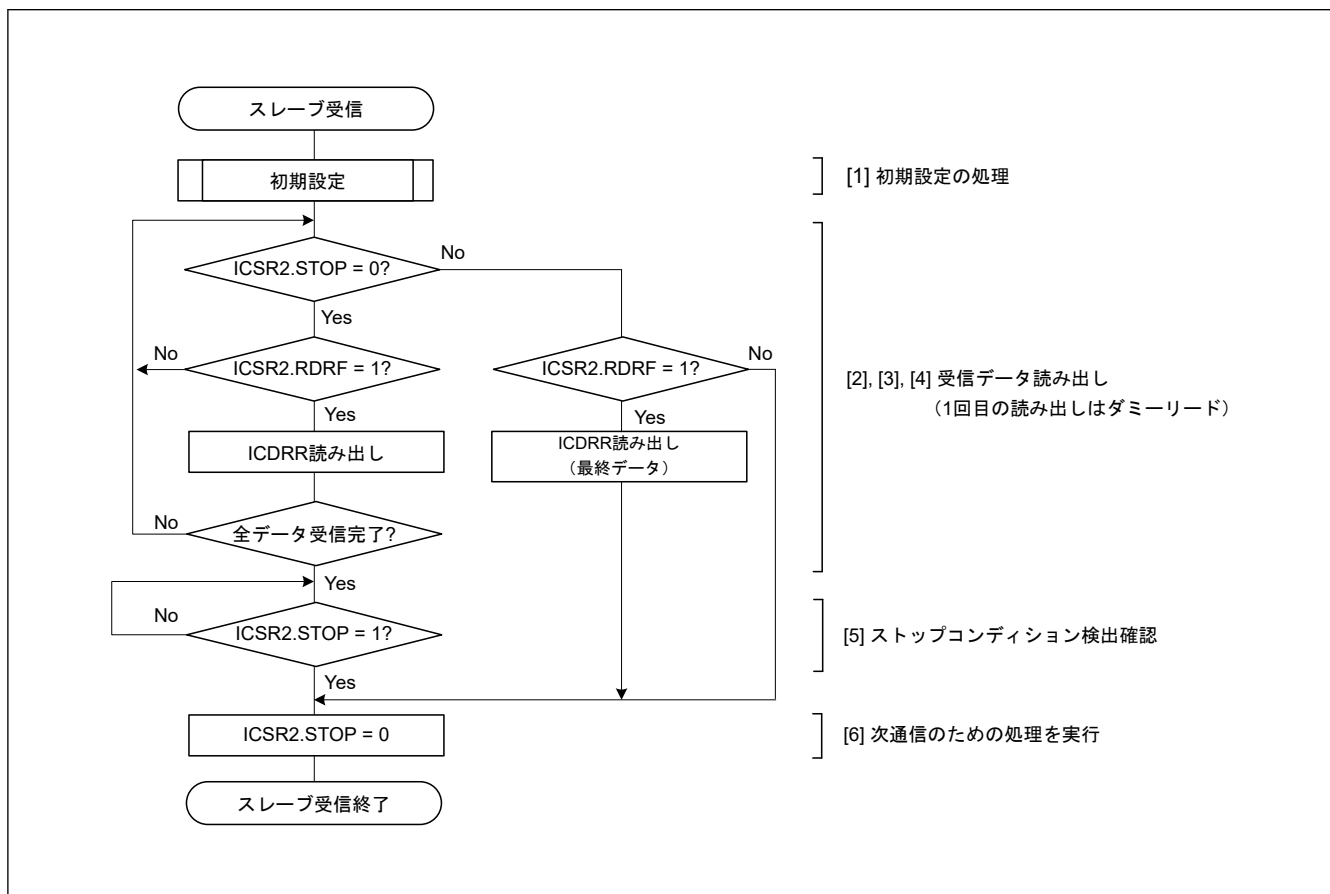
図 25.18 スレーブ受信のフローチャート例
