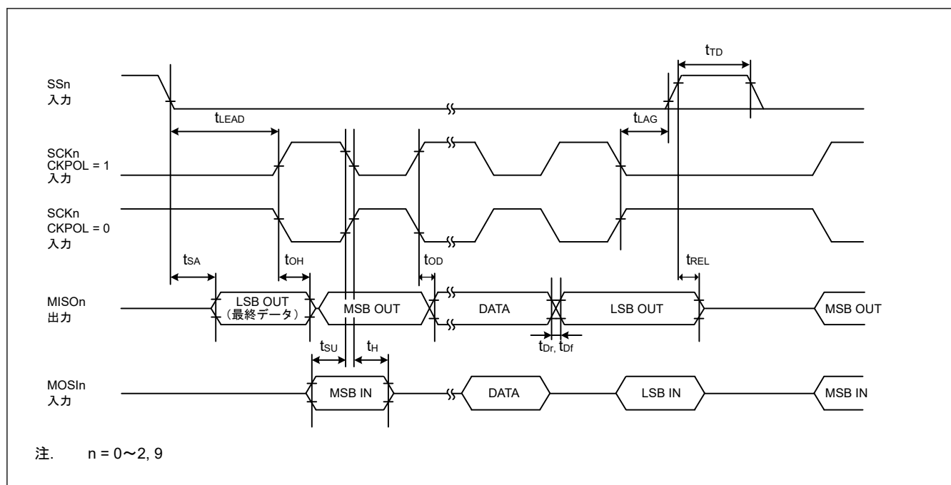
図 35.37 SCI 簡易 SPI モードタイミング (スレーブ、CKPH = 0)
