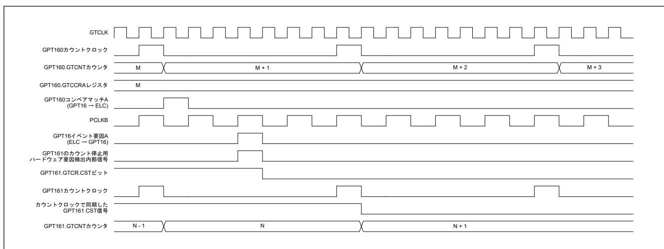
図 20.97 ELC_GPTA からのイベント入力に対応するカウントストップ動作のタイミング例
