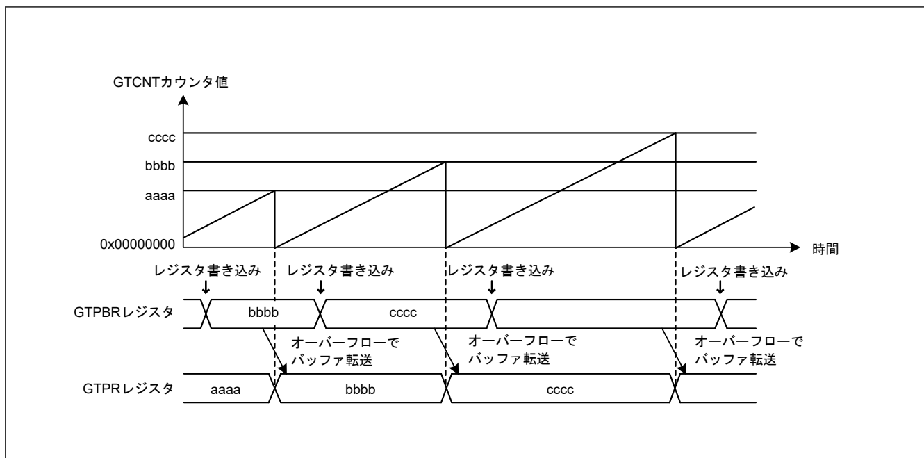
図 20.18 GTPR レジスタのバッファ動作例 (のこぎり波でアップカウントの場合)
