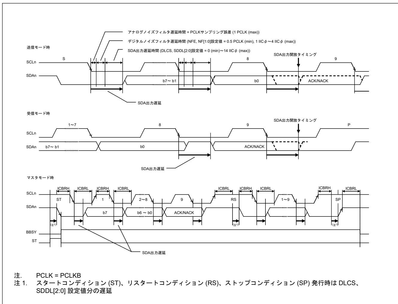
図 25.22 SDA 出力遅延機能
