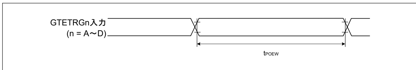
図 35.14 POEG 入力トリガタイミング
