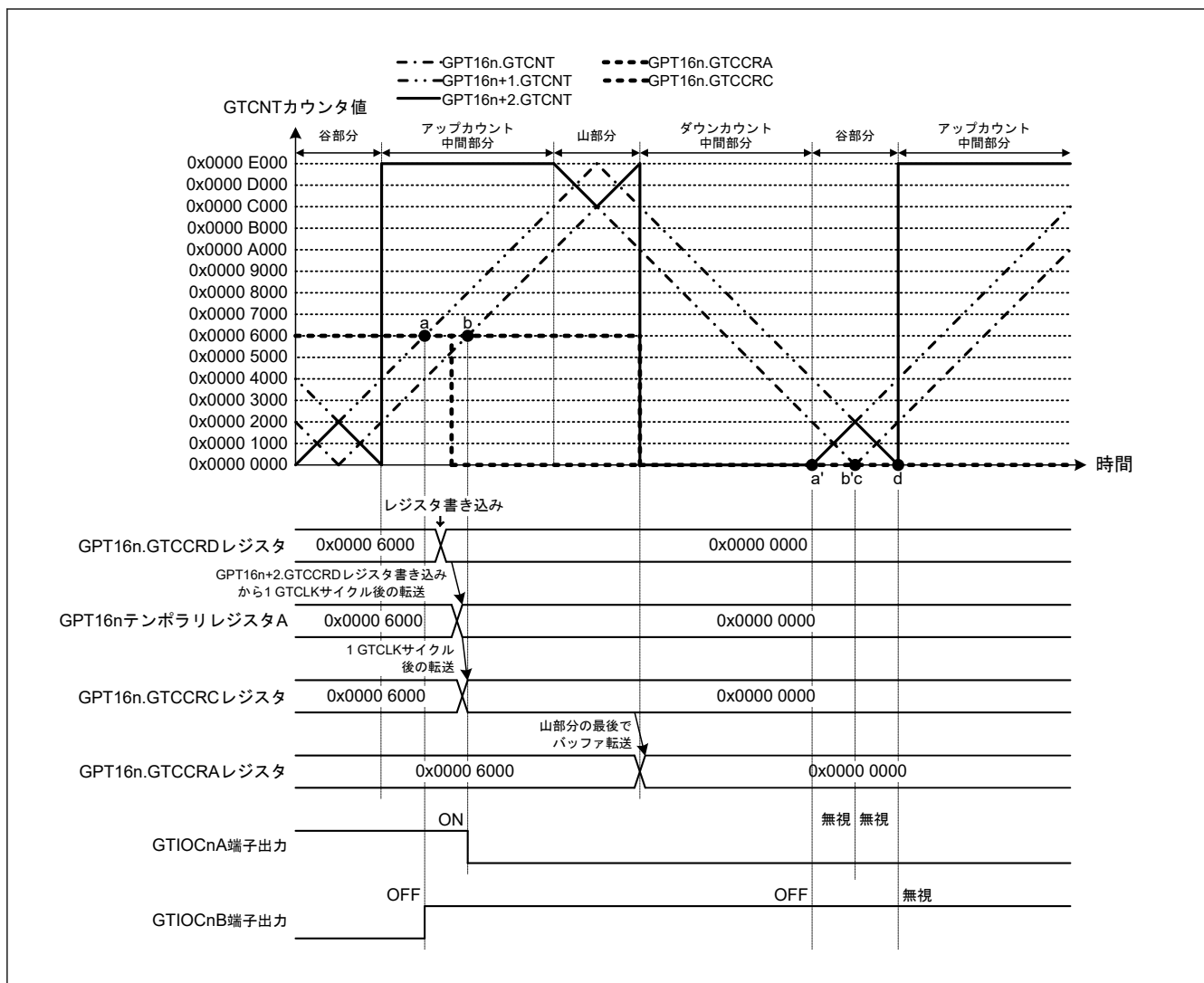
図 20.66 相補 PWM モードでのコンペアマッチ発生シーケンス動作例 (相補 PWM モード 3 シングルバッファ動作、アップカウントの GTCCRA レジスタコンペアマッチ時: GTIOcNA 端子 = Low/GTIOcNB 端子 = High、ダウンカウントの GTCCRA レジスタコンペアマッチ時: GTIOcNA 端子 = High/GTIOcNB 端子 = Low、デッドタイム値: 0x0000 2000、コンペアマッチ発生順序: a' → (b', c) → d) (n = 0)
