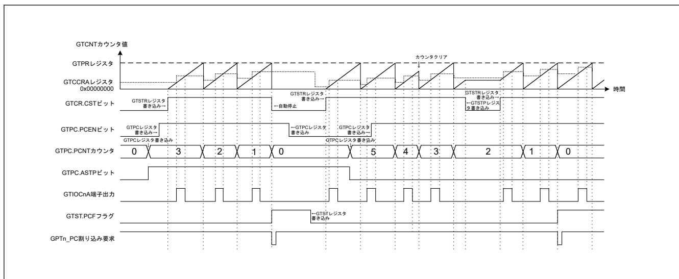
図 20.121 PWM 周期計数機能の例 (のこぎり波ワンショットパルスモード)
