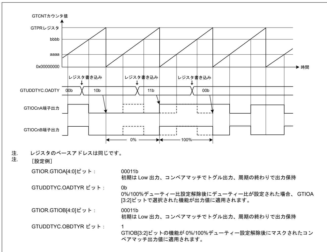
図 20.88 出力デューティ 0%、100%機能動作例
