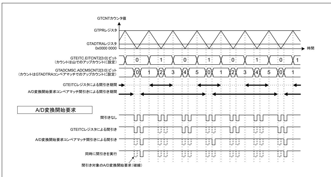
図 20.157 A/D 変換開始要求コンペアマッチ間引き機能の動作例 (拡張割り込み間引き : EIVTC2[1:0] = 01b、EADTAL[2:0] = 010b、A/D 変換開始要求コンペアマッチ間引き : ADCMSC2[1:0] = 01b、ADCMSC2[2:0] = 010b)
