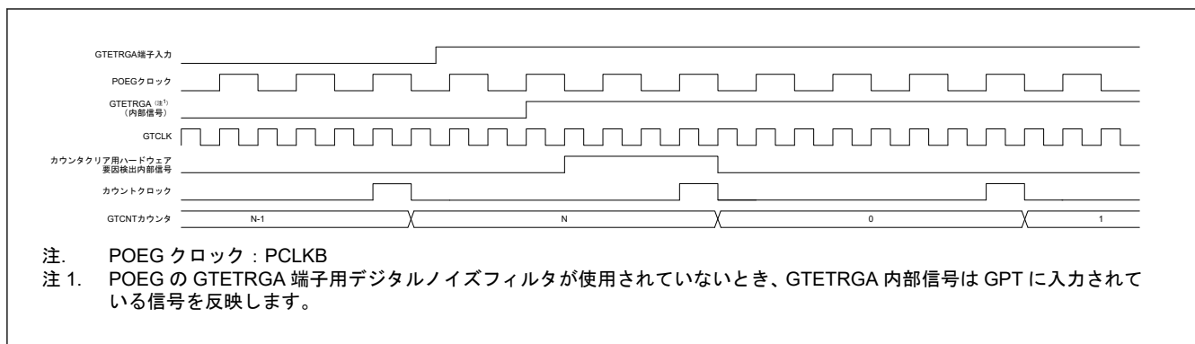
図 20.101 GTETRGA 端子入力の立ち上がりエッジに対応するカウンタクリアの動作タイミング例 (GTCLK 信号の分周により生成されるクロック信号の周期計数中)
