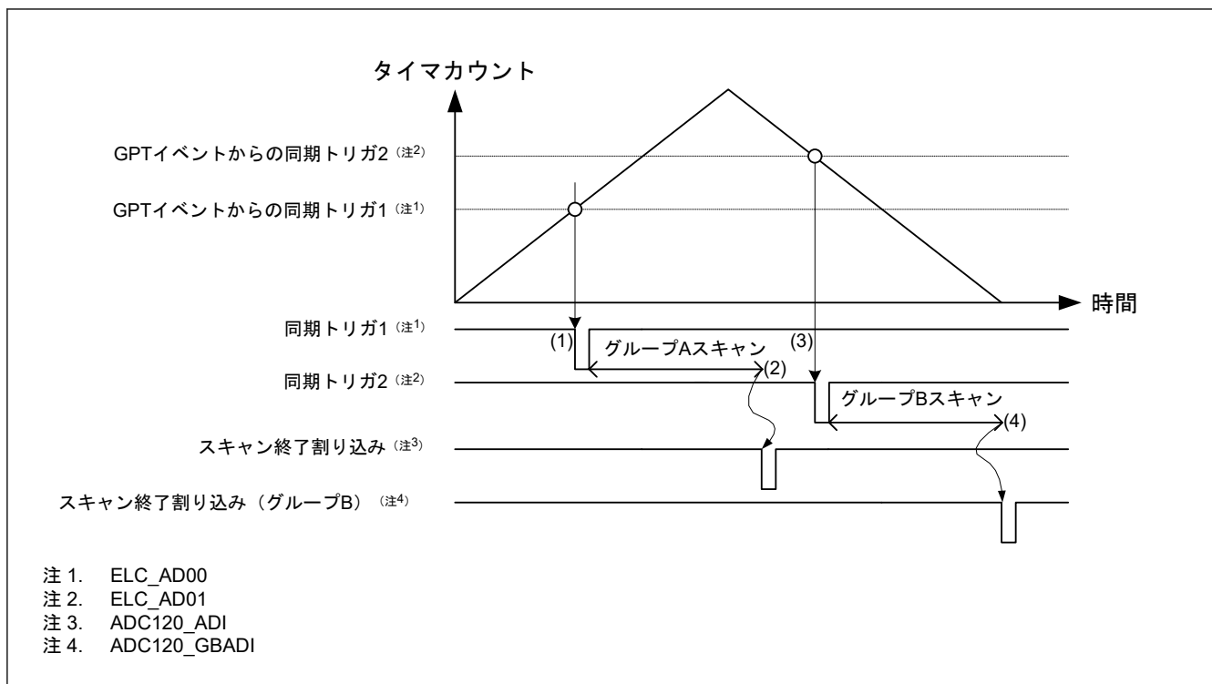
図 29.18 グループスキャンモードの基本動作例 (ELC からの同期トリガ使用)
