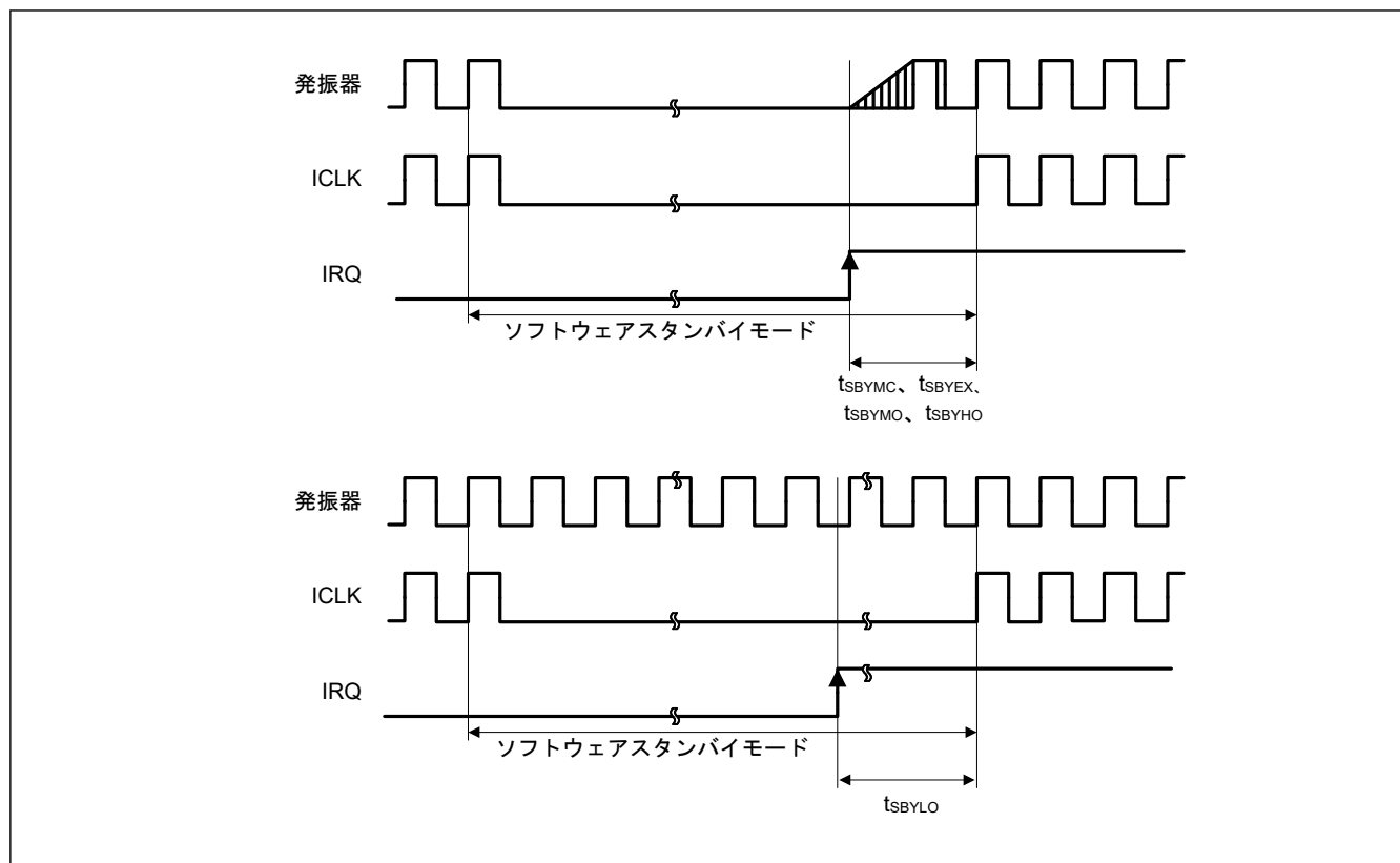
図 35.9 ソフトウェアスタンバイモード解除タイミング
