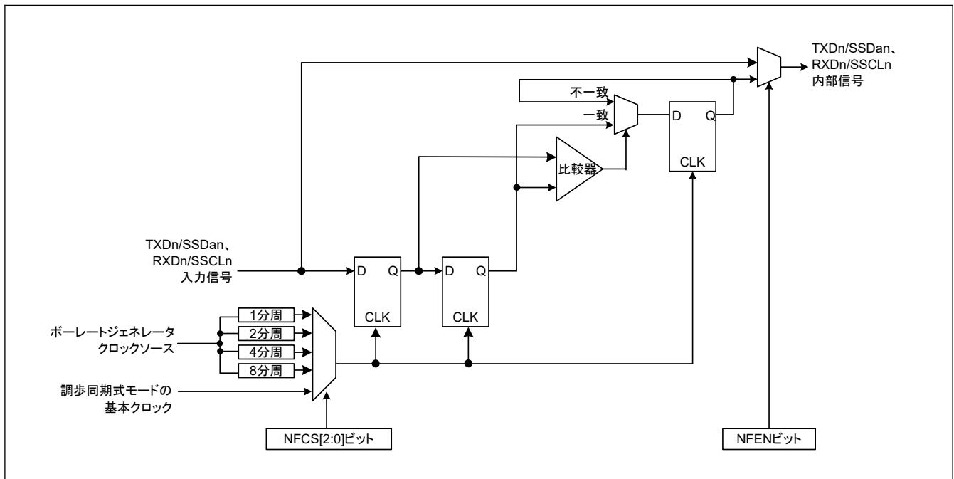
図 24.71 デジタルノイズフィルタ回路のブロック図
