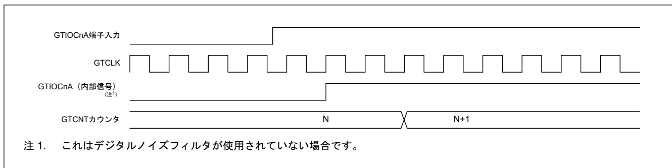
図 20.7 イベントカウント動作例 (GTIOCnA 端子入力の立ち上がりエッジによるアップカウント時)
