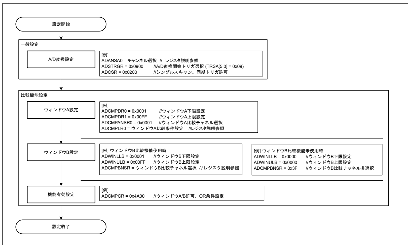
図 29.27 コンペア機能のイベント出力使用時の設定例
