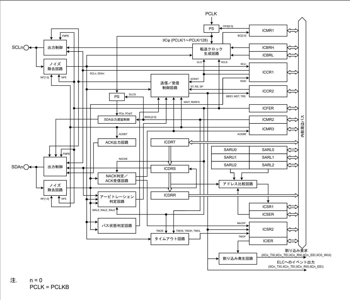
図 25.1 IIC のブロック図
