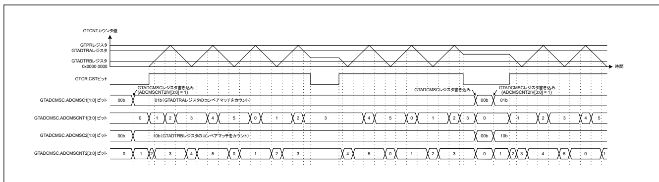
図 20.156 A/D 変換開始要求コンペアマッチ間引き機能の動作例
