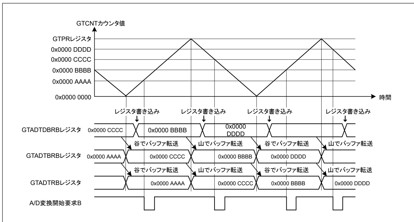
図 20.33 GTADTRA および GTADTRB レジスタのダブルバッファ動作例（三角波、谷と山の両方でバッファ転送、アップカウントとダウンカウントの両方で A/D 変換開始要求発生の場合）
