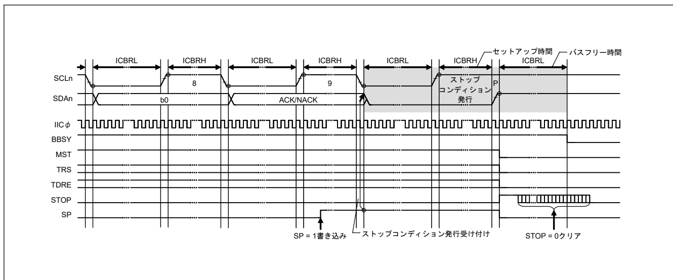
図 25.47 ストップコンディション発行タイミング (SP ビットの使用)
