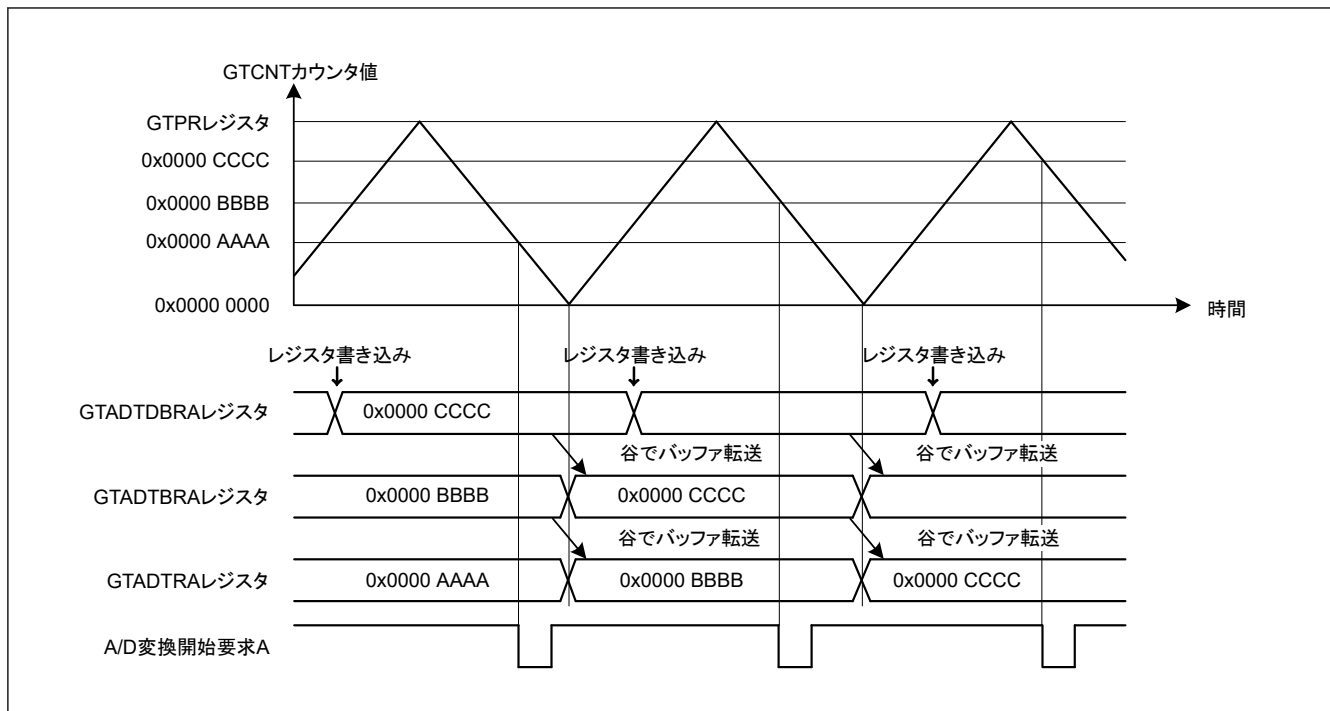
図 20.32 GTADTRA および GTADTRB レジスタのダブルバッファ動作例（三角波、谷でバッファ転送、ダウンカウントで A/D 変換開始要求発生の場合）
