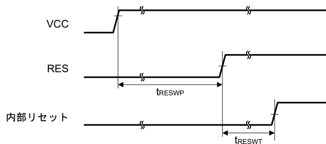
図 35.6 電源投入時リセット入力タイミング
