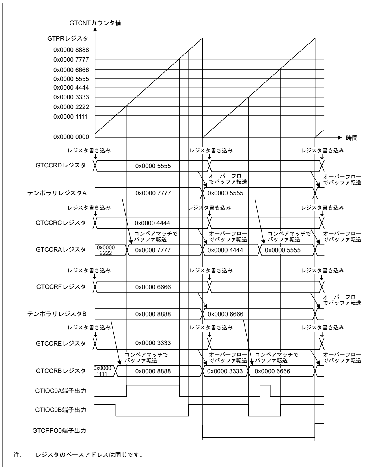
図 20.42 のこぎり波ワンショットパルスモードの動作例 (アップカウント、カウントスタート時に GTIOCnA 端子 = Low 出力/GTIOCnB 端子 = High 出力、GTCCRA/GTCCRB レジスタのコンペアマッチ時にトグル出力、周期の終わりで出力保持、GTIOR.PSYE = 1 の場合)
