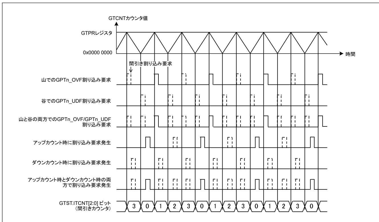
図 20.143 割り込み間引き機能の動作例（三角波、谷と山の両方をカウントして間引き、間引き回数 3、ダウンカウントで間引き開始の場合）
