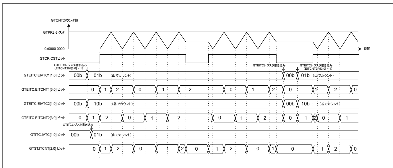
図 20.145 割り込み間引き用のカウンタ動作例
