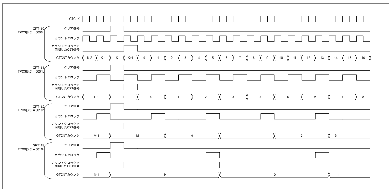
図 20.111 ソフトウェアによる同時クリアの動作例 (異なるカウント周期)
