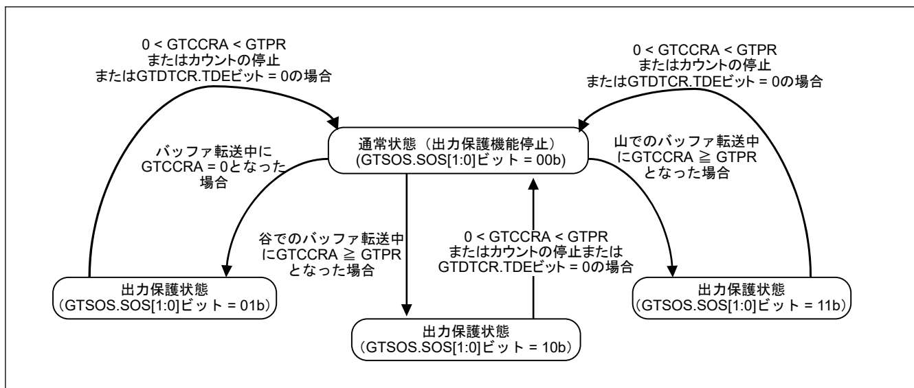
図 20.171 出力保護機能
