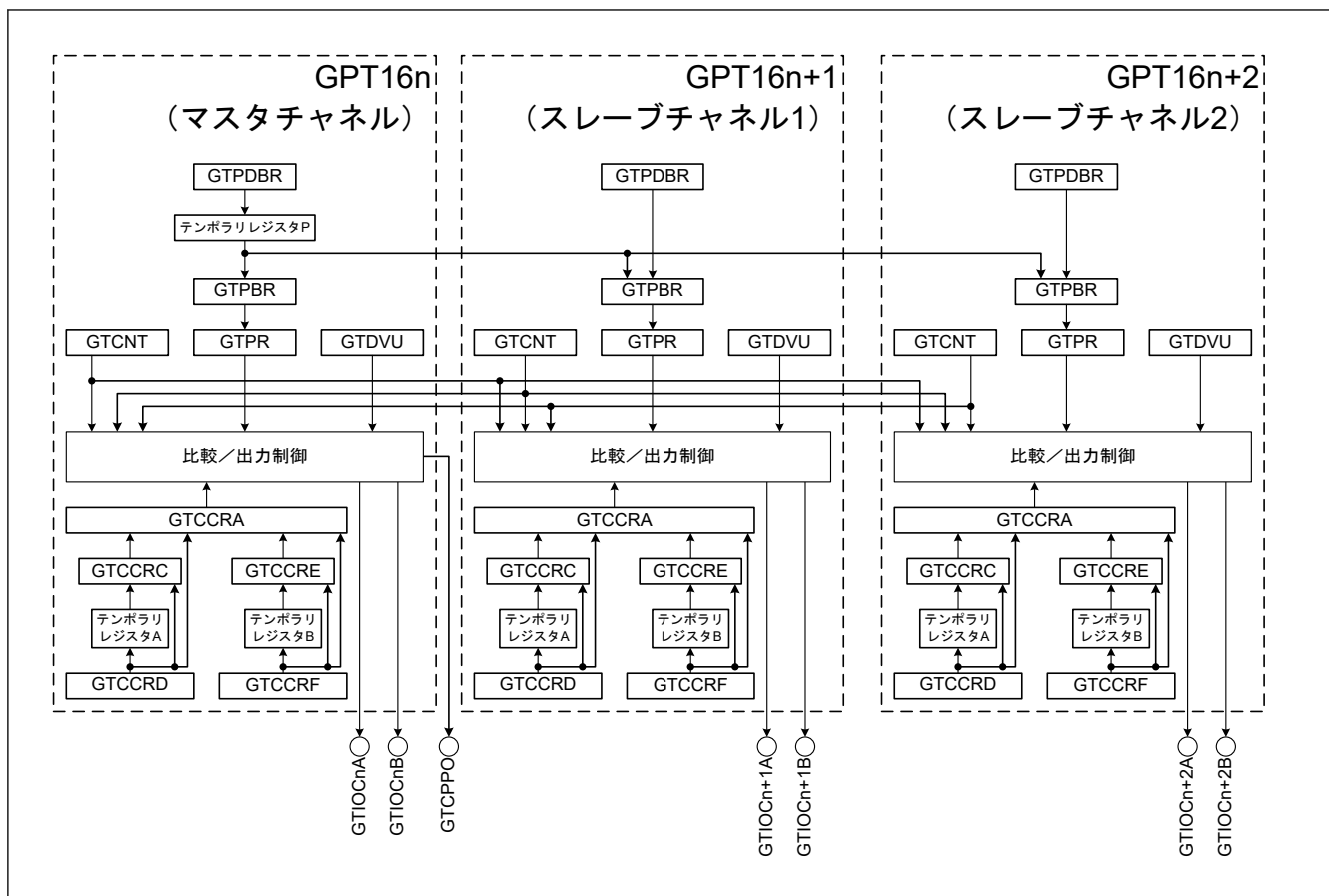
図 20.69 相補 PWM モード 4 のブロック図 (n = 0)
