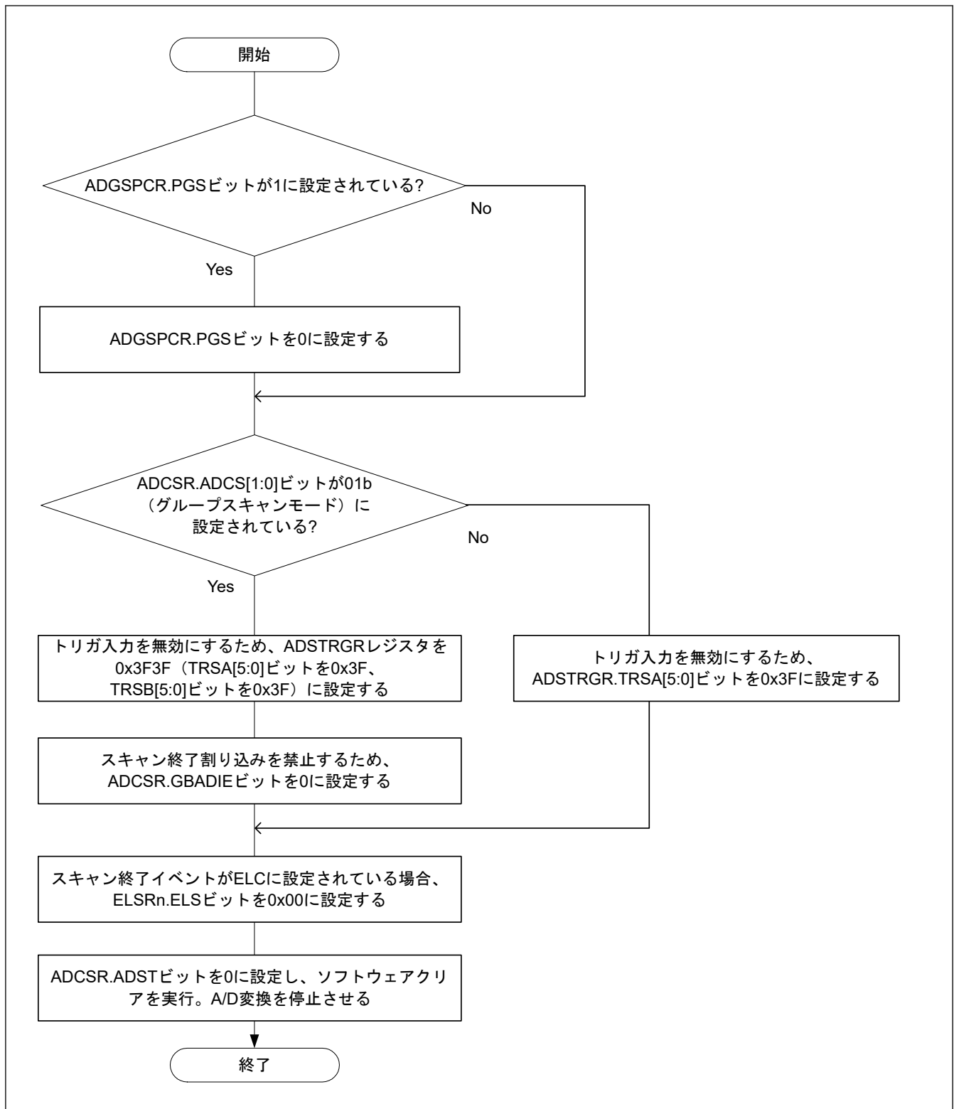
図 29.36 ソフトウェアによる ADCSR.ADST ビットのクリア手順
