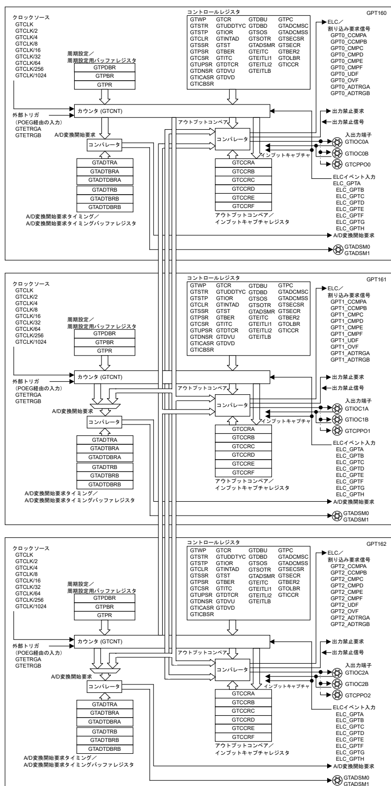
図 20.2 GPT のブロック図 (のこぎり波 PWM モード 1、2、のこぎり波ワンショットパルスモード、三角波 PWM モード 1、2、3、相補 PWM モード 1、2、3、4)
