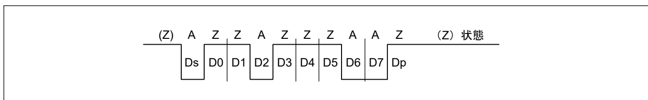
図 24.49 ダイレクトコンベンション (SCMR.SDIR ビット = 0、SCMR.SINV ビット = 0、SMR_SMCI.PM ビット = 0)
