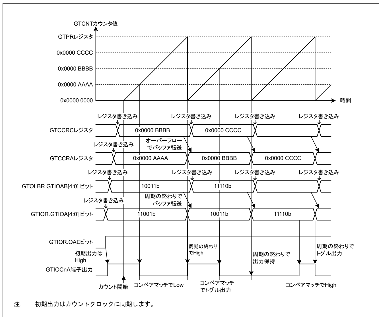
図 20.35 GTIOA ビットおよび GTIOB ビットのバッファ操作例 (のこぎり波 PWM モード1 のアップカウント、周期の終わりにバッファ転送)
