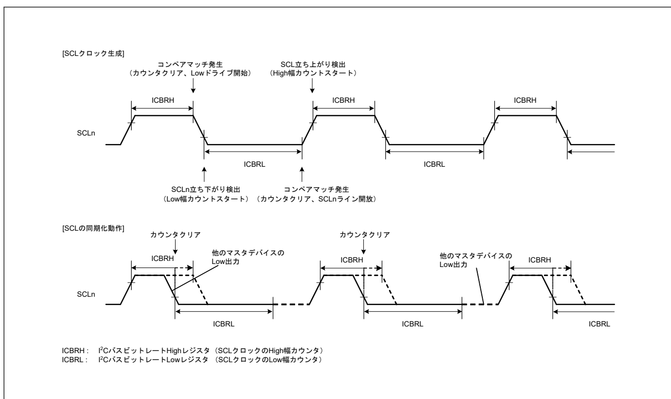
図 25.21 IIC の SCL クロック生成および SCL 同期化動作
