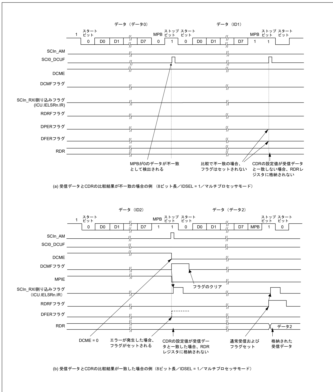
図 24.6 アドレス一致検出の例 (2) (マルチプロセッサモード)
