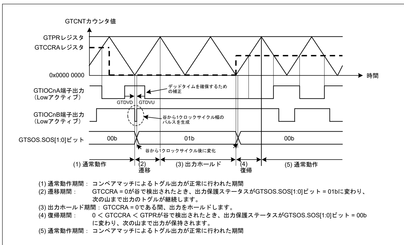
図 20.174 山のバッファ転送中に GTCCRA レジスタが 0x0000 0000 になったときの出力保護機能の動作例 (谷でのバッファ転送中に 0 < GTCCRA < GTPR に復帰、アクティブレベルは : Low) ( n = 0 \sim 2 )
