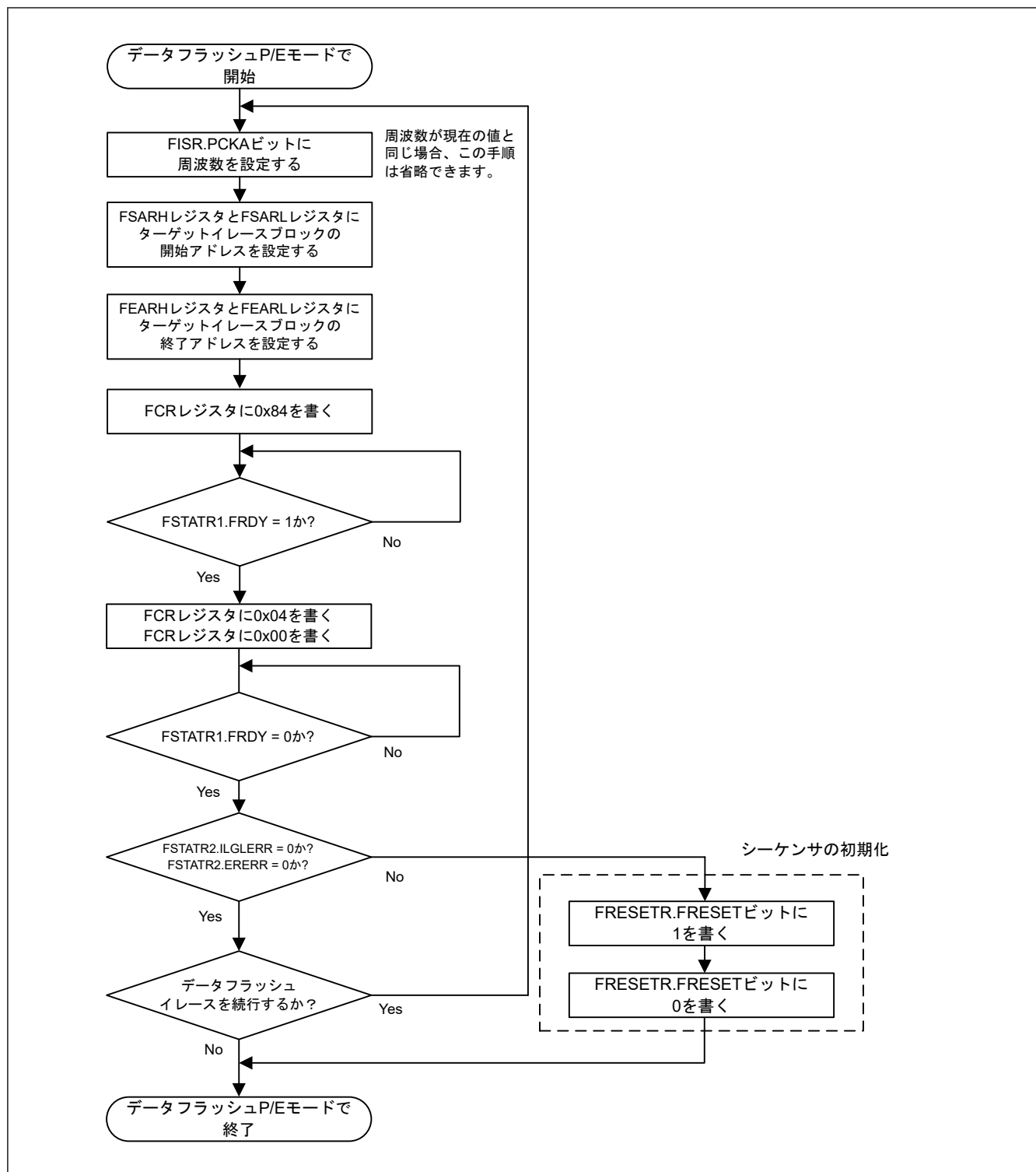
図 33.24 データフラッシュブロックイレース手順のフローチャート
