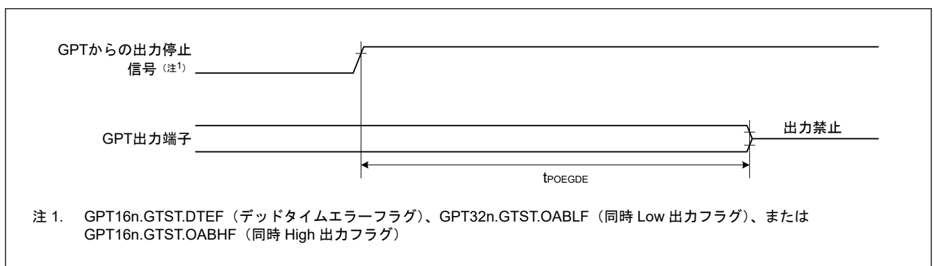
図 35.16 GPT からの出力停止信号の検出に対応した POEG の出力禁止時間
