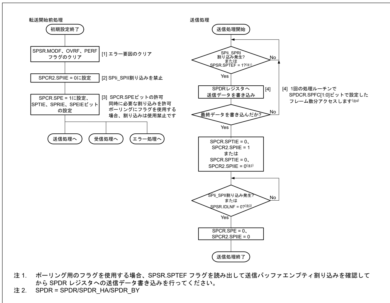
図 26.36 スレーブモードでの送信フロー
