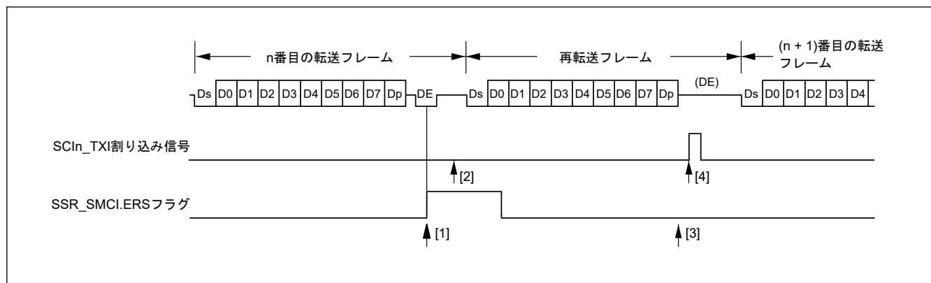
図 24.52 スマートカードインタフェース送信モードでのデータ再送信動作
