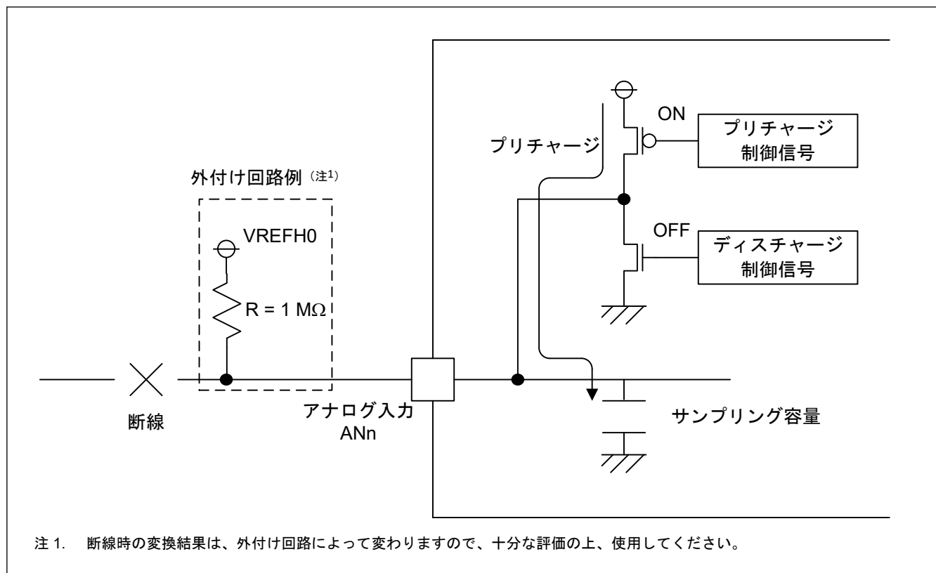
図 29.32 プリチャージを選択した場合の断線検出例
