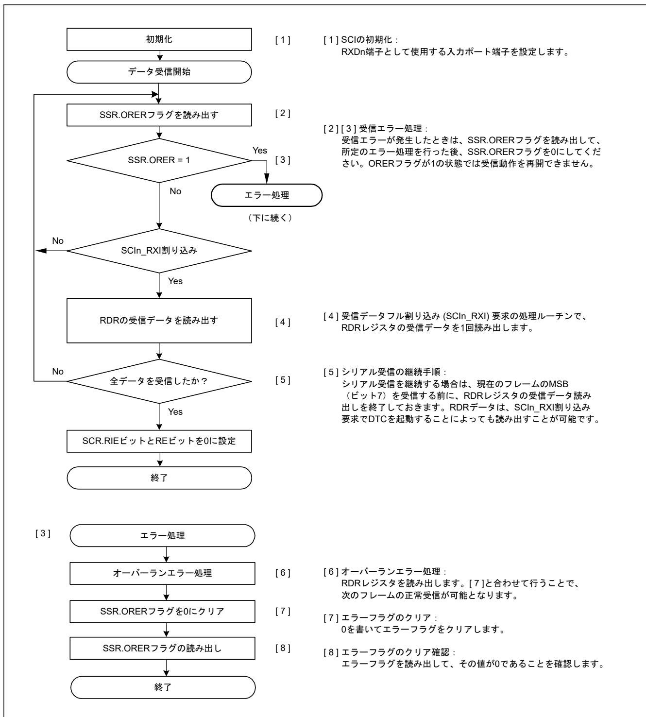
図 24.43 クロック同期式モードにおけるシリアル受信のフローチャート例 (非 FIFO 選択時)
