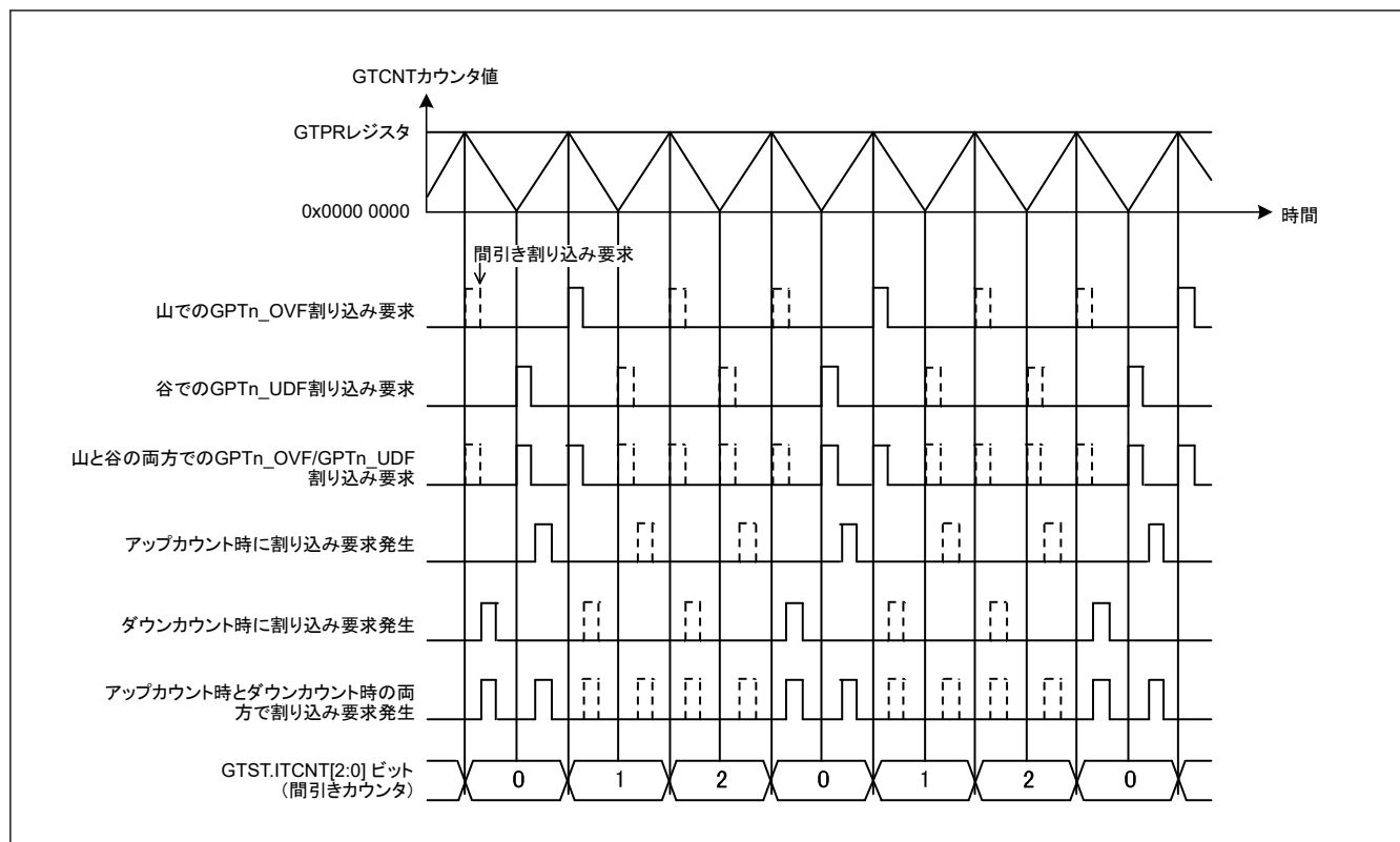
図 20.139 割り込み間引き機能の動作例（三角波、山をカウントして間引き、間引き回数 2 の場合）
