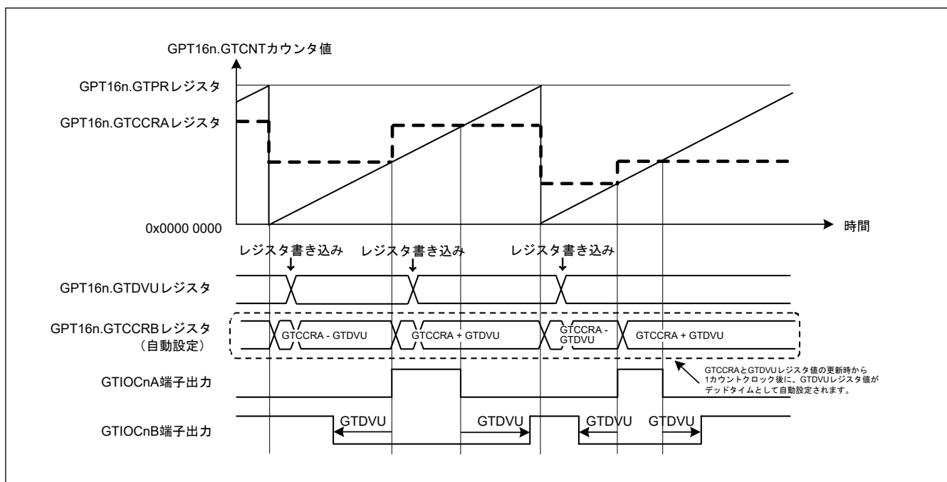
図 20.80 デッドタイム自動設定機能の動作例 (のこぎり波ワンショットパルスモード、アップカウント、GPT163 でアクティブ High の場合)
