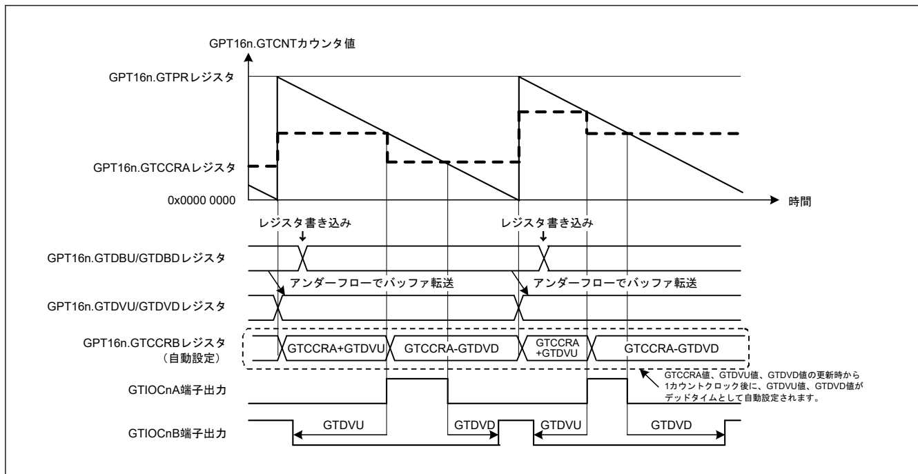
図 20.81 デッドタイム自動設定機能の動作例 (のこぎり波ワンショットパルスモード、ダウンカウント、GTDVU と GTDVD はバッファ動作に設定、GPT160～GPT162 でアクティブ High の場合)
