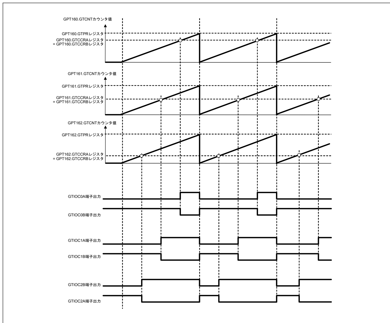
図 20.116 のこぎり波 3 相相補 PWM 出力例
