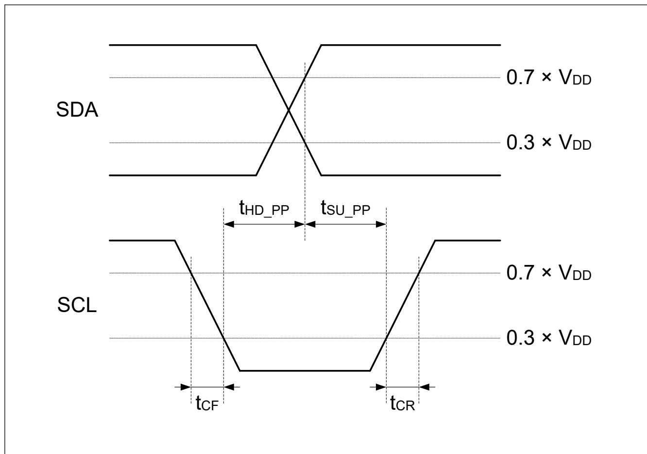
図 36.38 I3C マスタ出力タイミング
