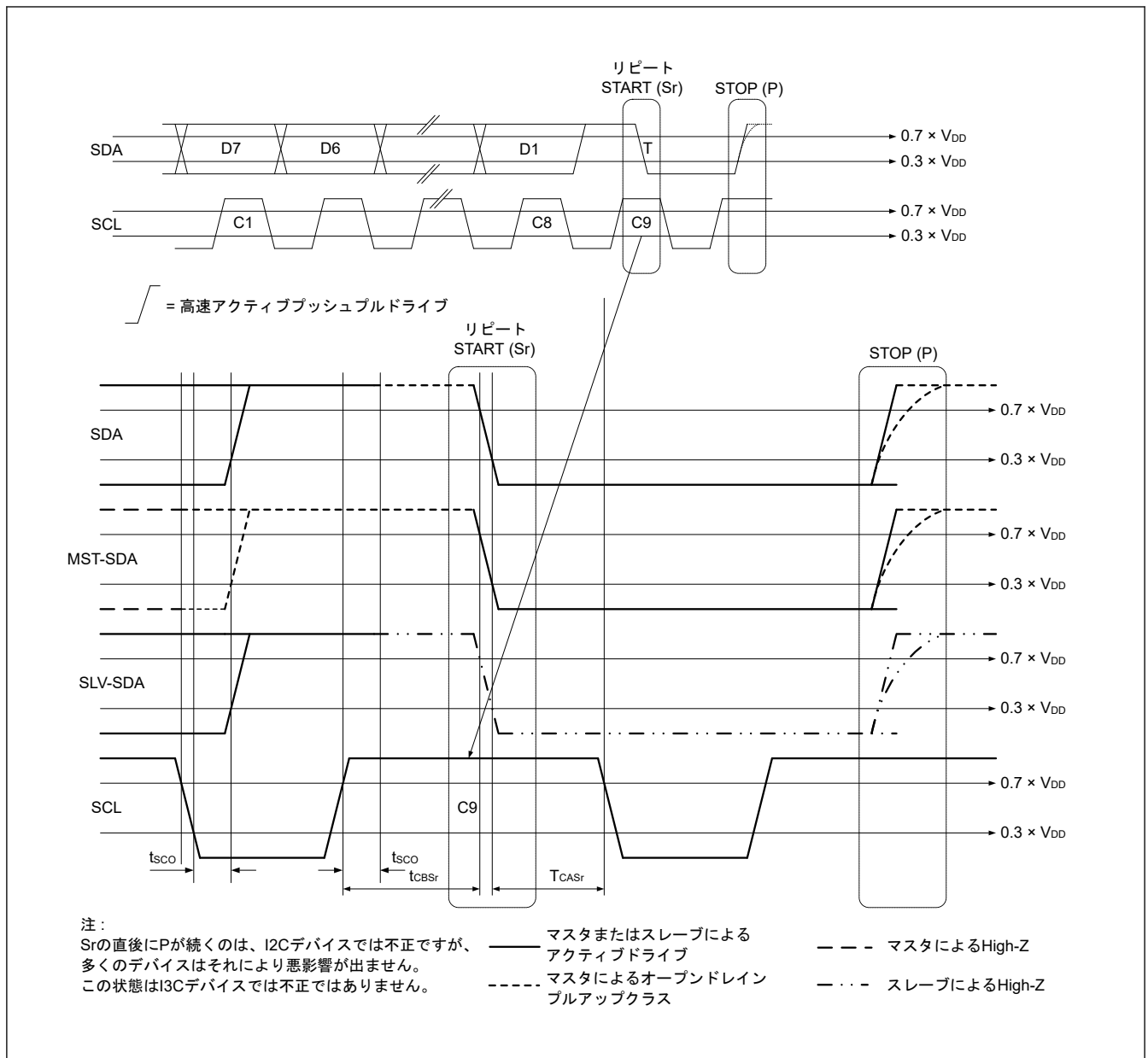
図 36.41 繰り返しのスタートコンディションおよびストップコンディションでのマスタ終了時の T ビット読み出し
