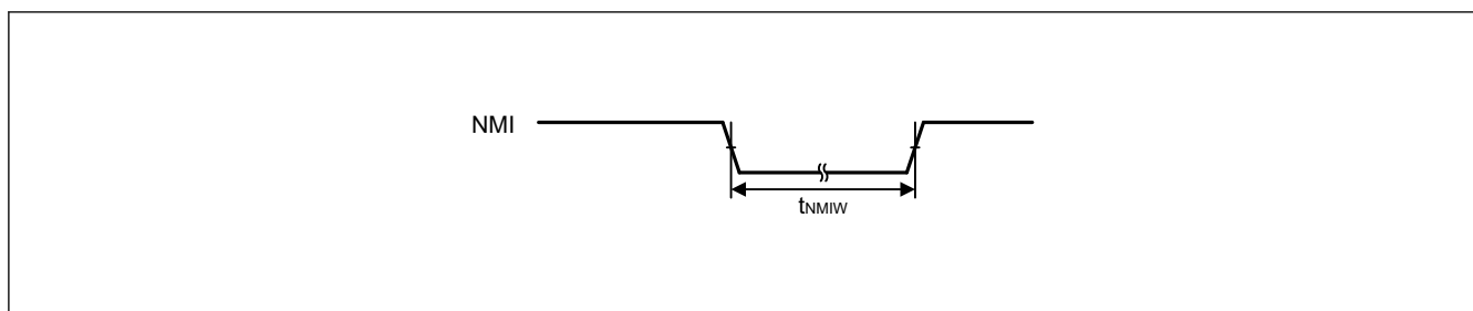
図 36.10 NMI 割り込み入力タイミング
