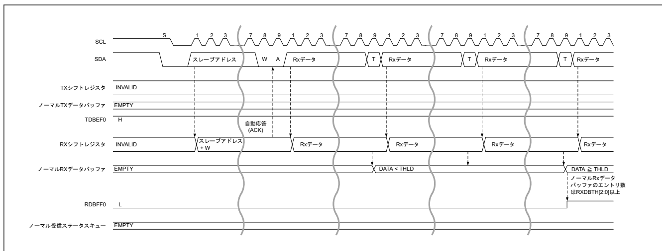
図 25.36 SDR データ書き込み転送タイミング (1/2)
