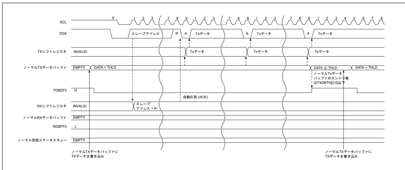
図 25.42 レガシー I2C メッセージデータ読み出し転送タイミング (1/2)
