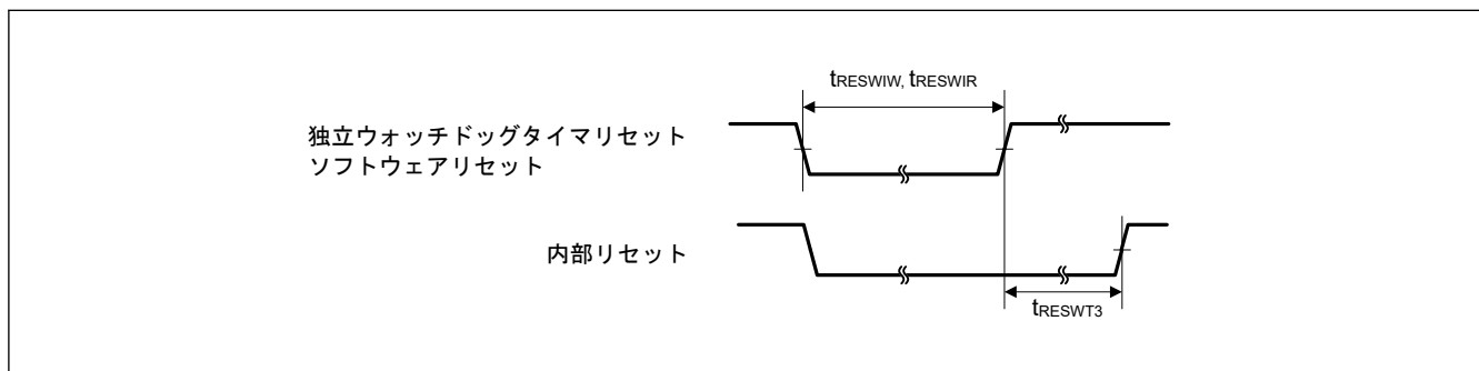
図 36.7 リセット入力タイミング (2)
