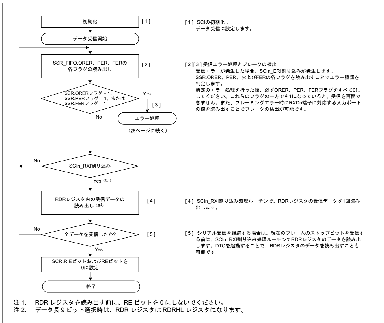
図 24.13 調歩同期式モードにおけるシリアル受信のフローチャート例（アドレス一致検出無効時）(1)
