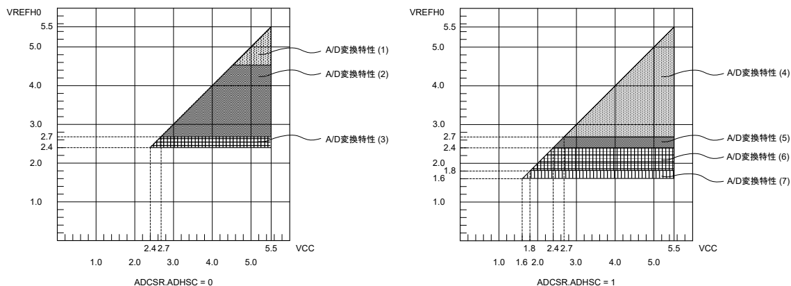
図 36.44 VCC0~VREFH0 電圧範囲
