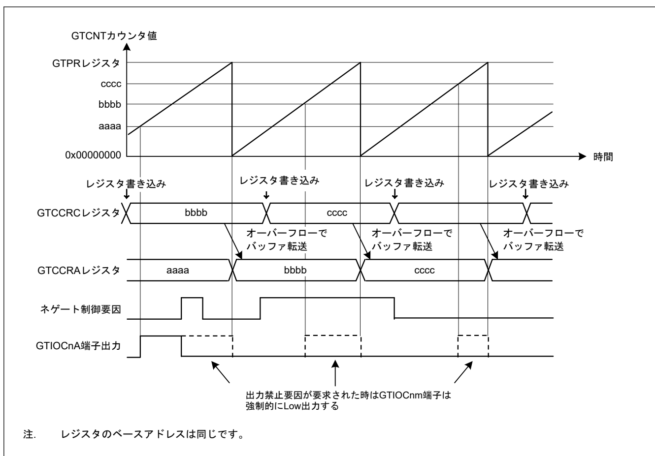
図 20.61 GTIOCnm 端子出力禁止制御動作例 (のこぎり波でアップカウント、バッファ動作、アクティブレベル 1、GTCCR レジスタのコンペアマッチで High 出力、周期の終わりで Low 出力、出力禁止で Low 出力の場合) (n = 4~9, m = A, B)
