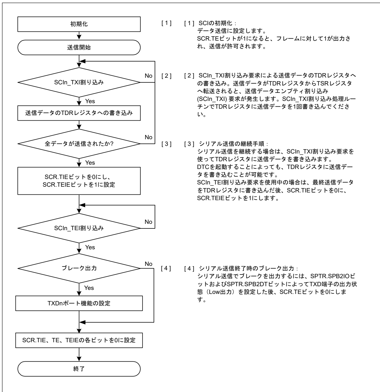
図 24.10 調歩同期式モードにおけるシリアル送信のフローチャート例
