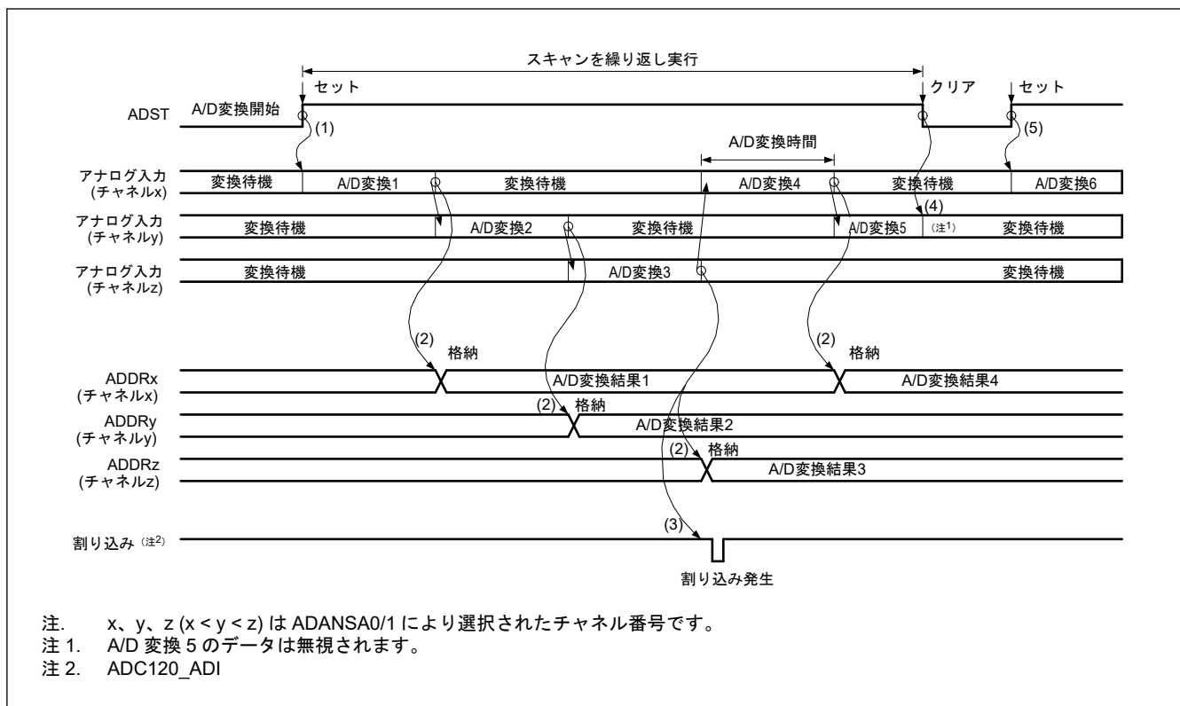
図 28.12 連続スキャンモードの基本動作例（アナログ入力（チャンネル x~z）選択）
