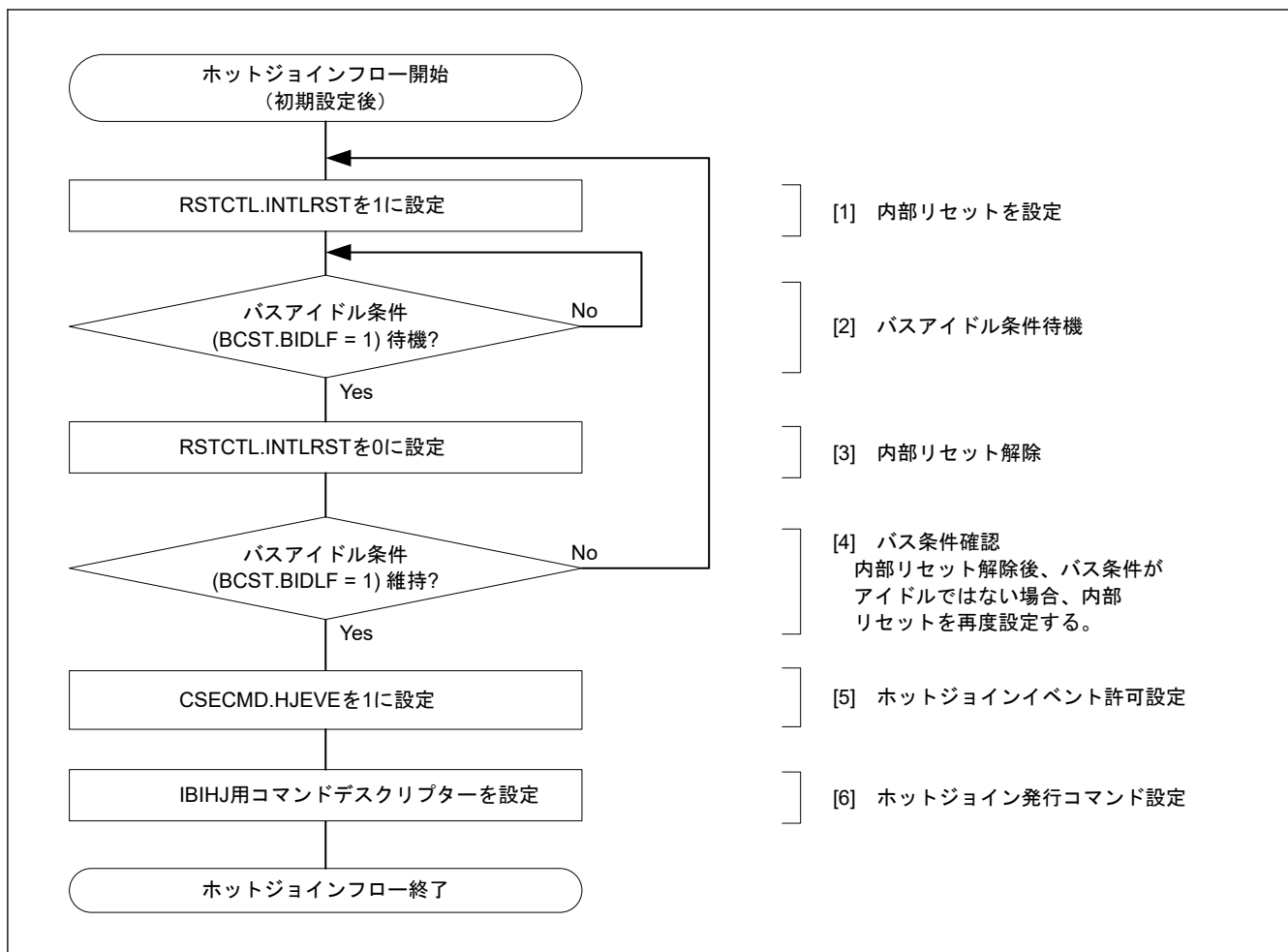
図 25.118 I3C バスがすでに設定済である場合のホットジョインのフローチャート
