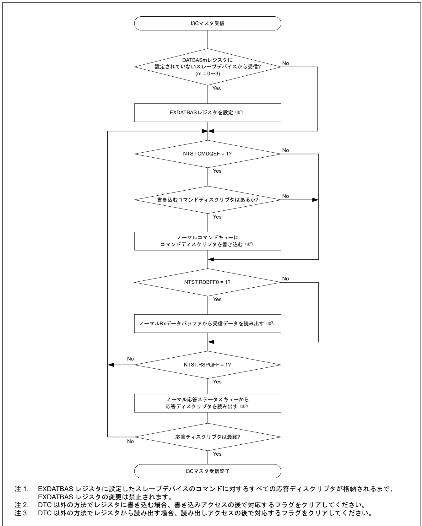
図 25.110 I3C マスタ受信のフローチャート例 (通常 FIFO バッファ転送)
