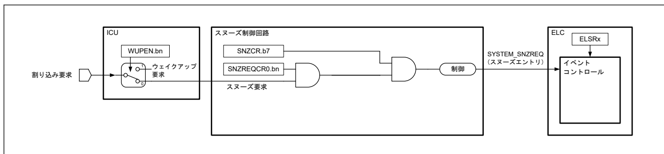
図 10.7 スヌーズモードエントリの構成
