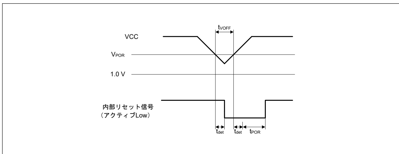
図 36.47 電圧検出しリセットタイミング
