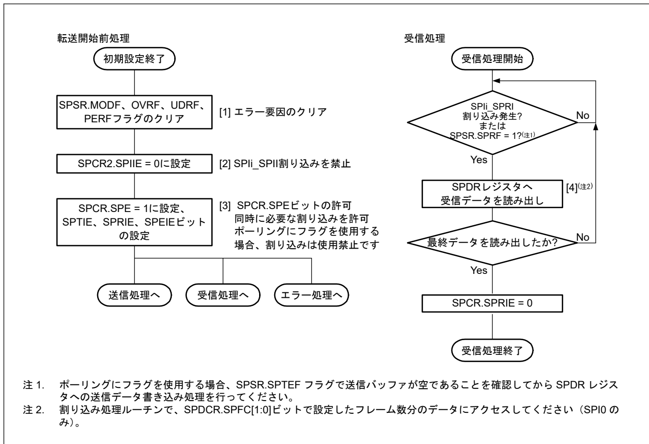
図 26.36 スレーブモードでの受信フロー
