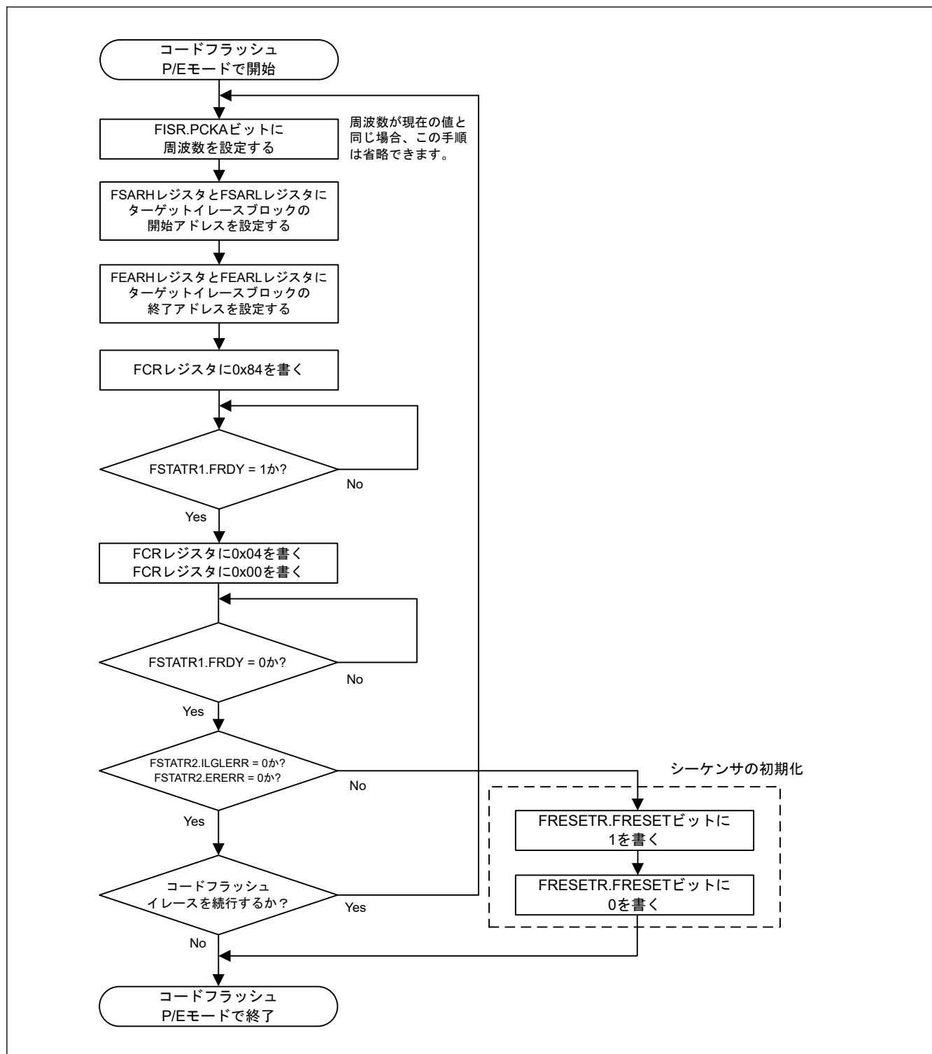
図 32.23 コードフラッシュブロックイレース手順のフローチャート
