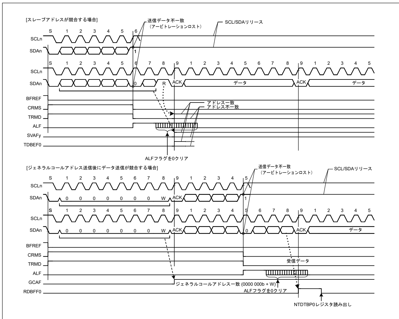
図 25.65 マスタアービトレーションロスト検出動作例 (MALE = 1 の場合)
