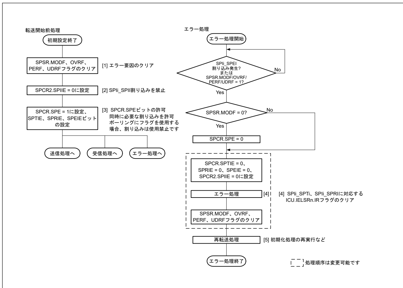
図 26.37 スレープモードでのエラー処理フロー
