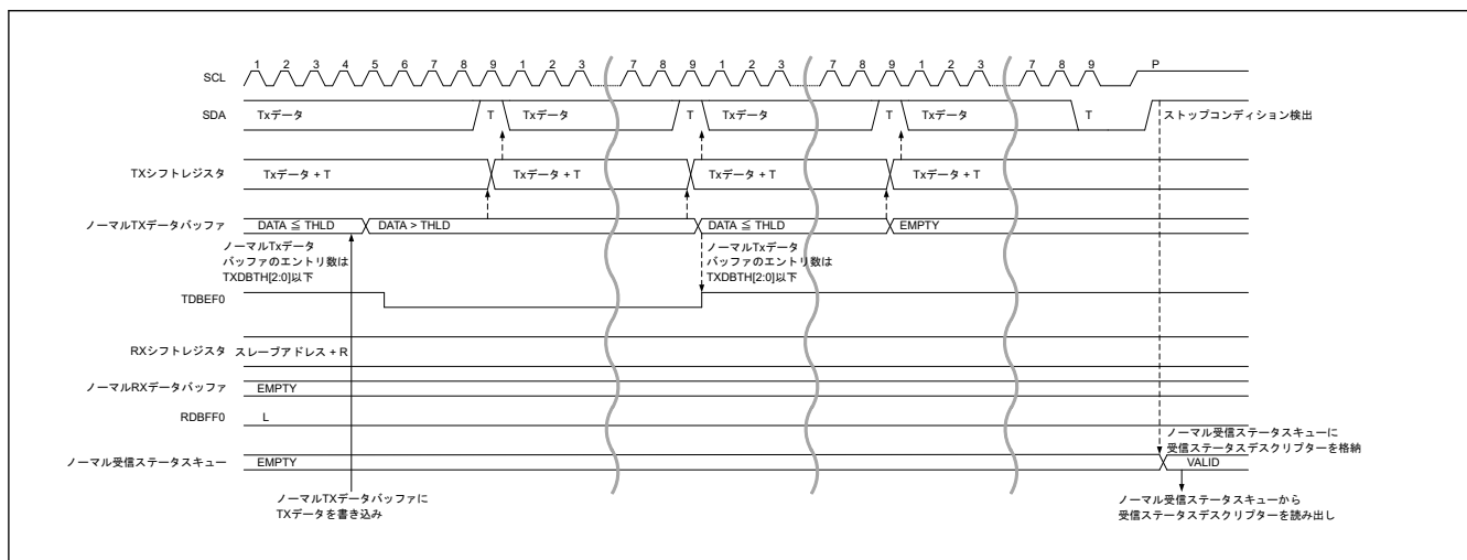
図 25.41 SDR データ読み出し転送タイミング (2/2)
