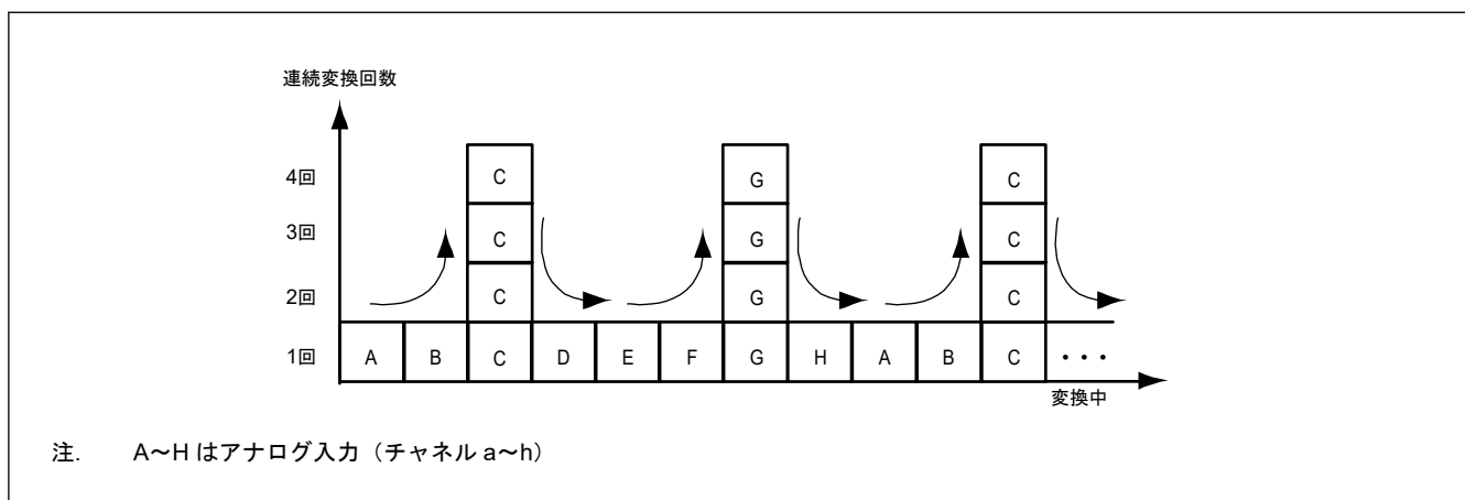
図 28.2 ADADC.ADC[2:0] = 011b および ADADS0/1 によるアナログ入力 C と G を 1 に選択時のスキャン変換シーケンス
