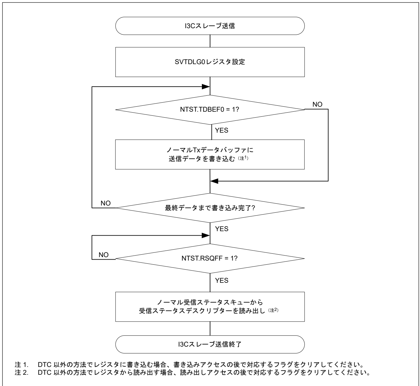
図 25.114 I3C スレーブ送信のフローチャート例 (通常 FIFO バッファ転送)
