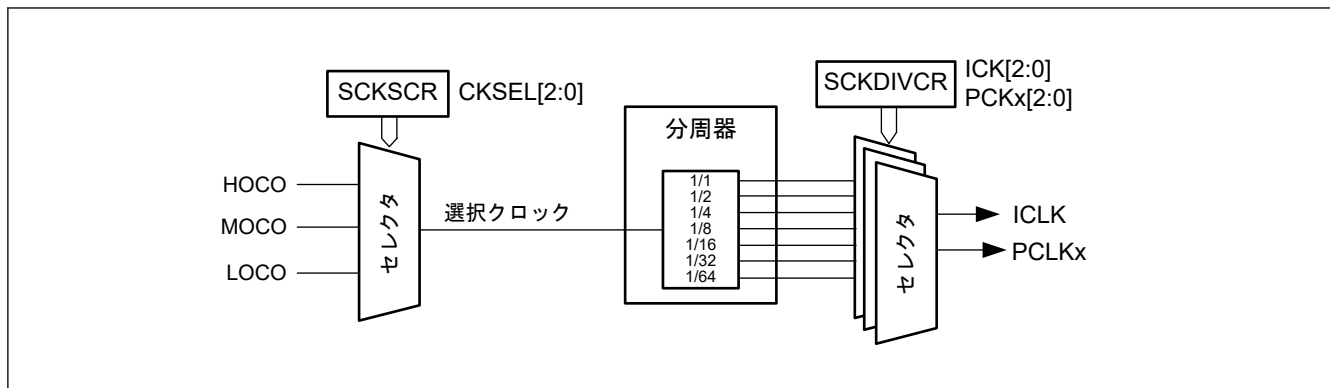
図 8.5 クロックソースセクタのブロック図
