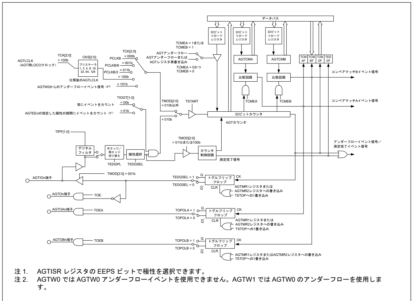
図 21.1 AGTW のブロック図
