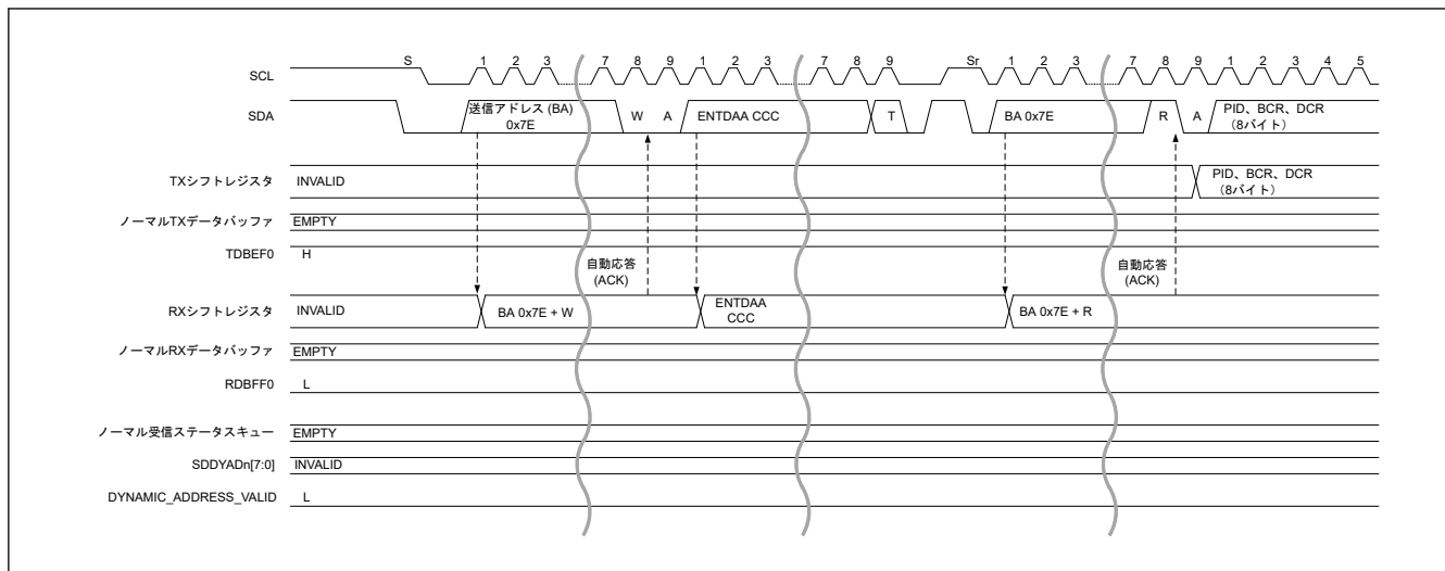
図 25.32 ダイナミックアドレス配置手順 (ENTDAA CCC) タイミング (1/3)
