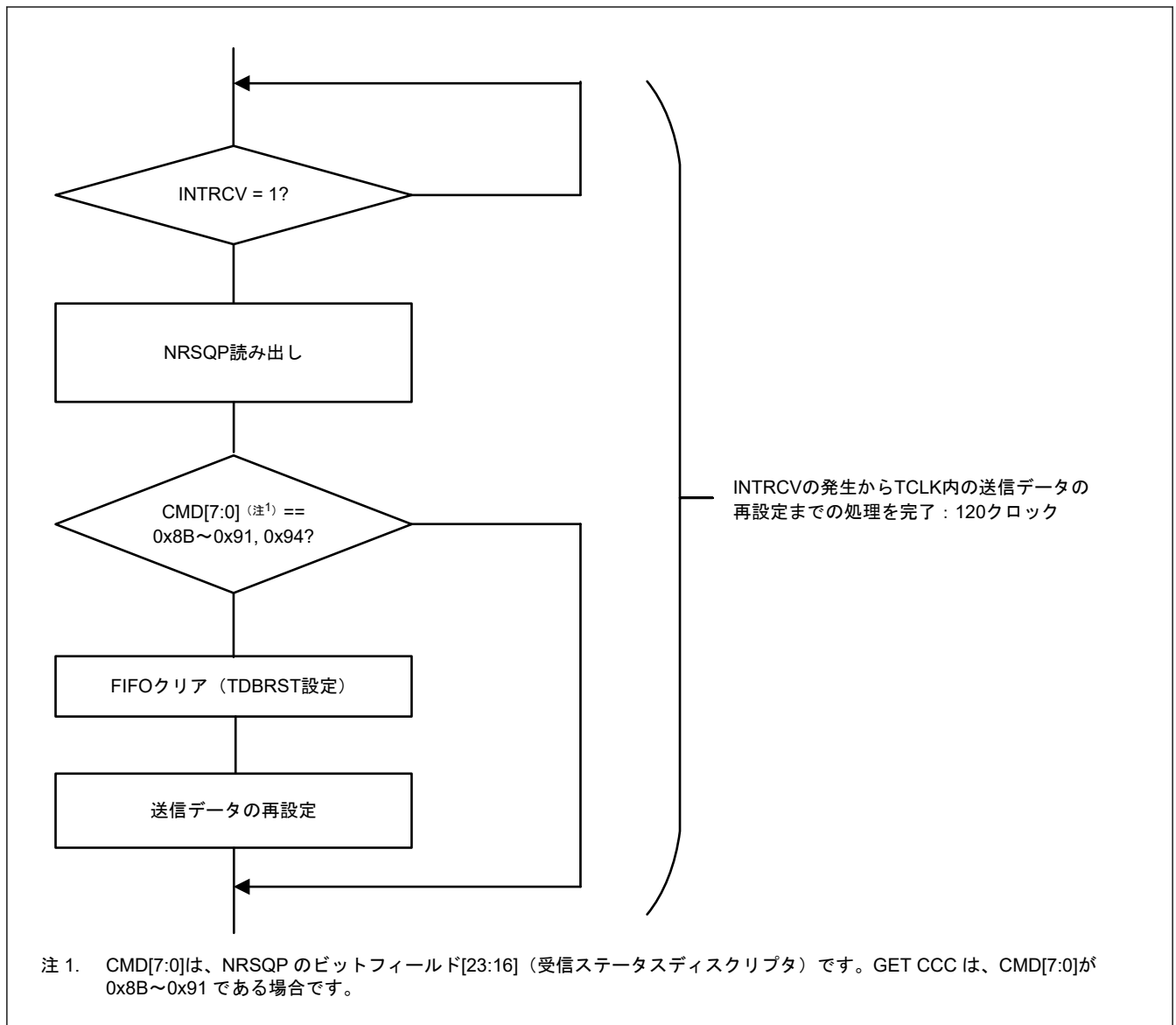
図 25.115 NDTBP0 レジスタから送信バッファへの書き込みによりデータが存在している間に I3C スレーブが GET CCC を受信する
