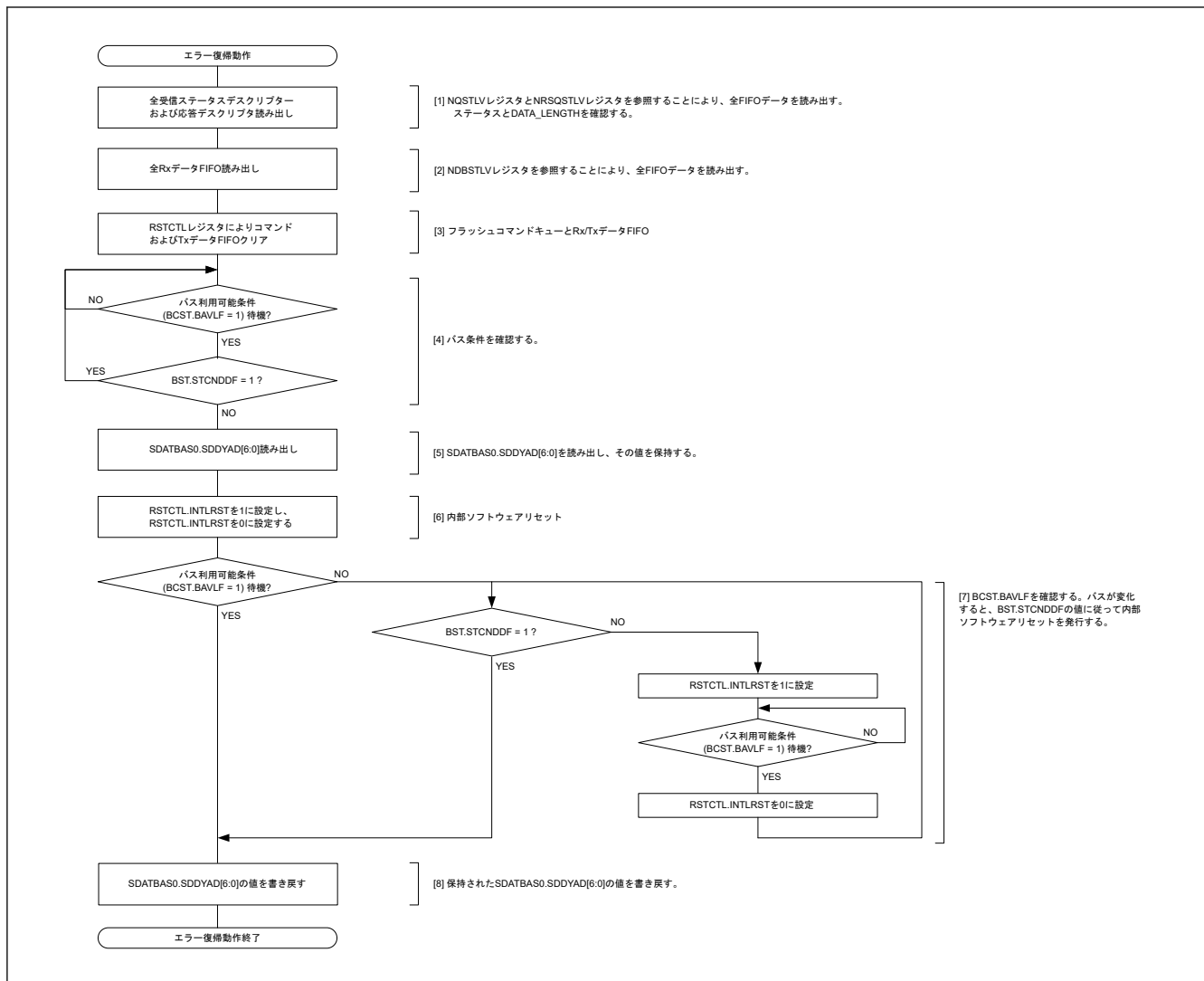
図 25.97 I3C スレーブのエラー復帰動作フローの例
