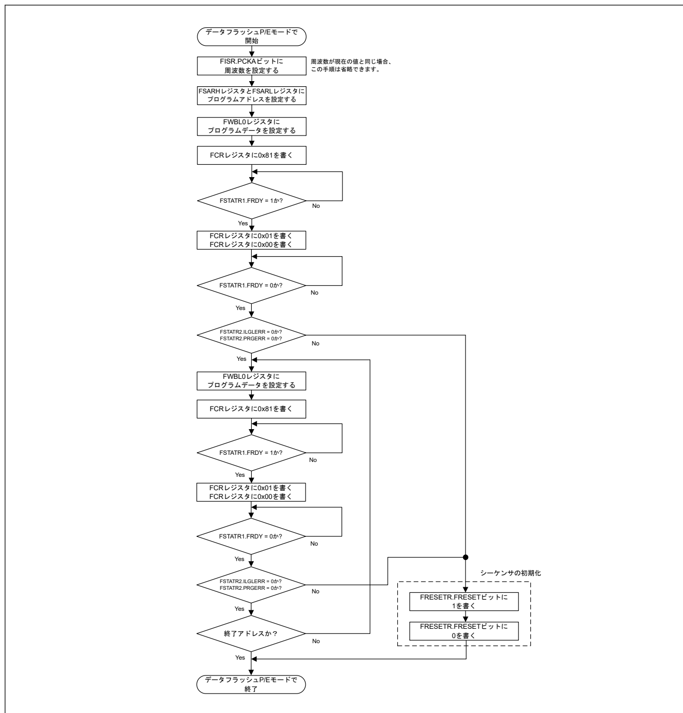
図 32.22 データフラッシュの連続プログラム時のフローチャート
