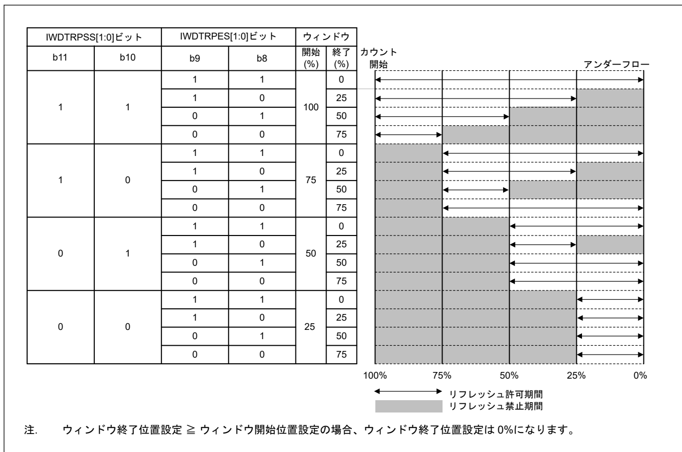
図 23.2 IWDTRPSS[1:0]ビットおよびIWDTRPES[1:0]ビットの設定とリフレッシュ許可期間
