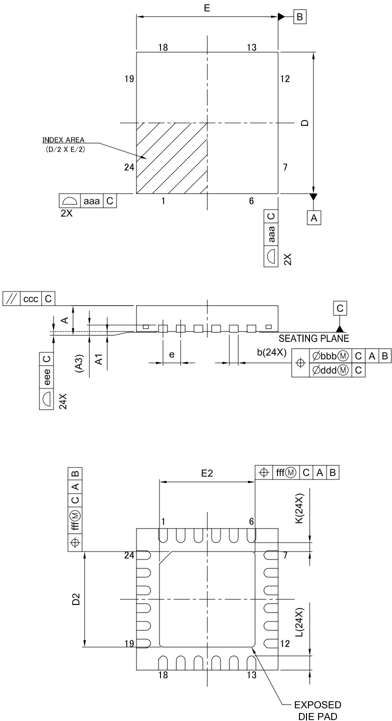
図 A2.1 HWQFN 24 ピン
