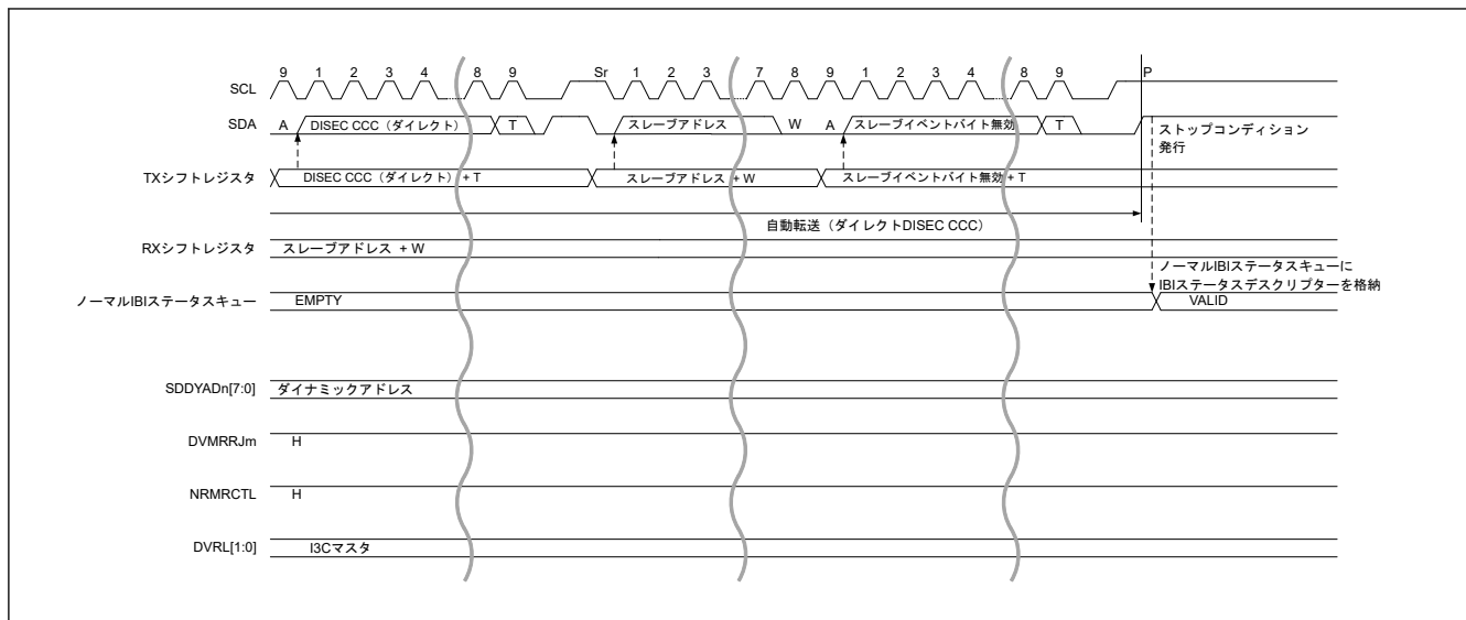
図 25.87 バス権要求 : NACK (DVMRRJ が 1) かつ NRMCTL が 1 の場合 (2/2)
