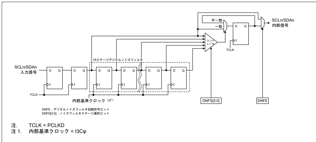
図 25.102 デジタルノイズフィルタ回路のブロック図
