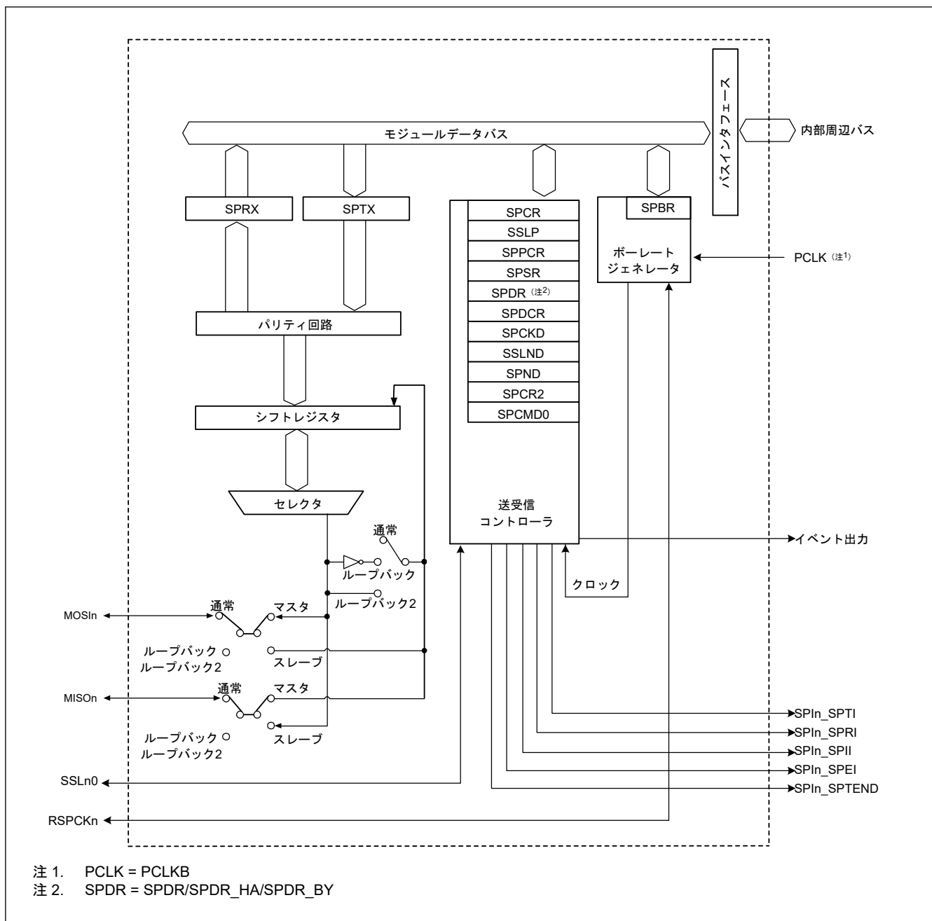
図 26.1 SPI のブロック図
