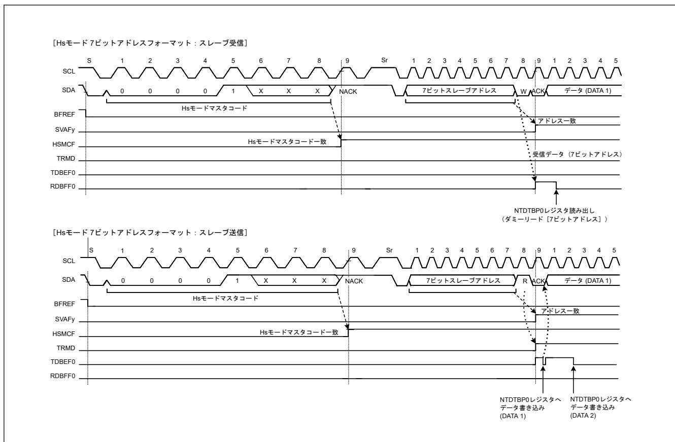
図 25.64 Hs モードマスタコード受信時に SVAfY/HSMCF フラグが1になるタイミング
