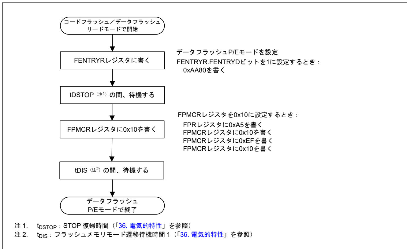
図 32.16 リードモードからデータフラッシュ P/E モードに切り替える手順
