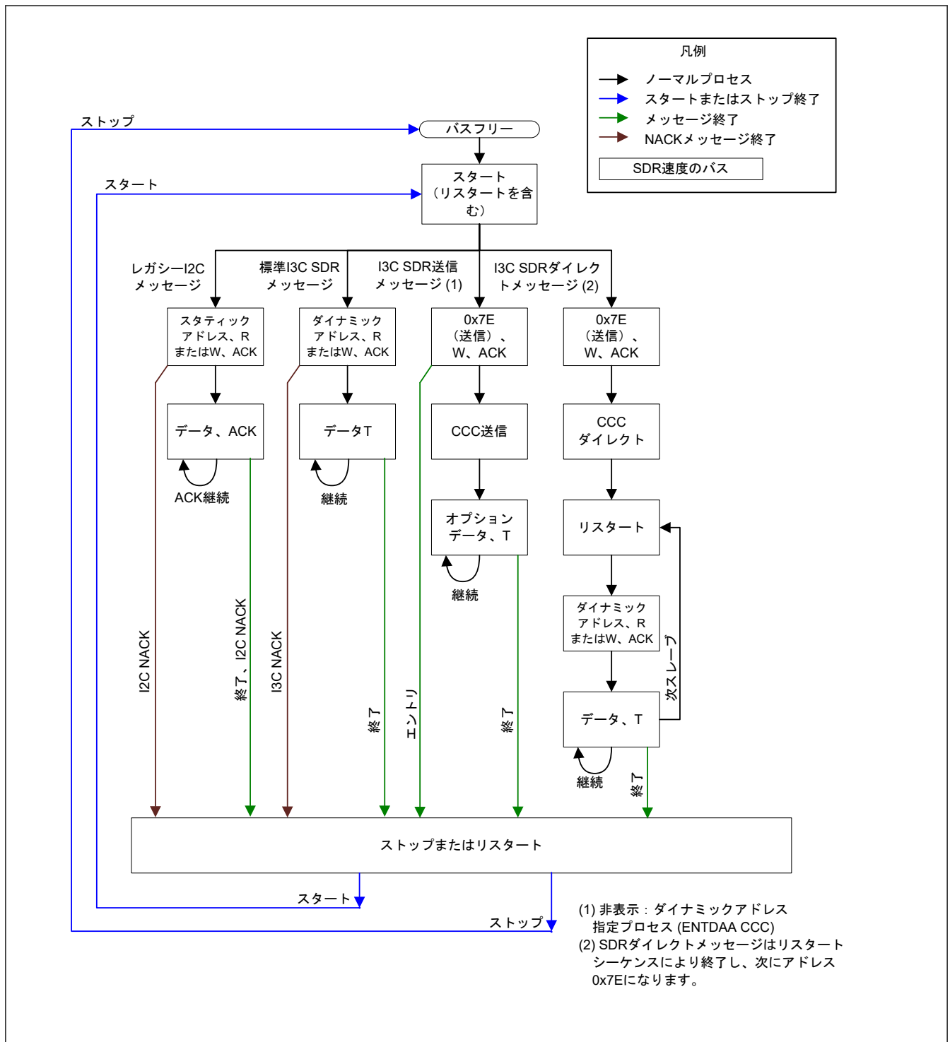
図 25.105 I3C 通信フロー
