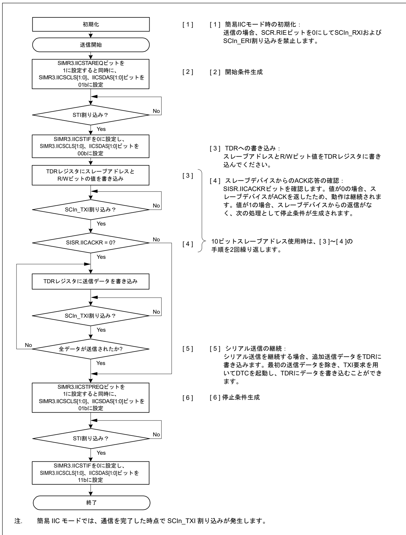
図 24.50 簡易 IIC モードにおけるマスタ送信のフローチャート例（送信割り込み、受信割り込み使用時）
