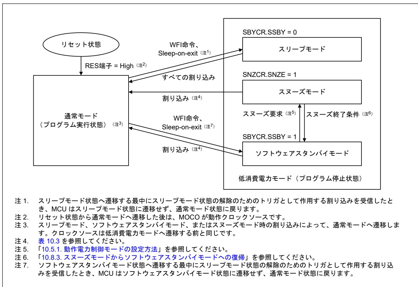
図 10.1 低消費電力モードの遷移
