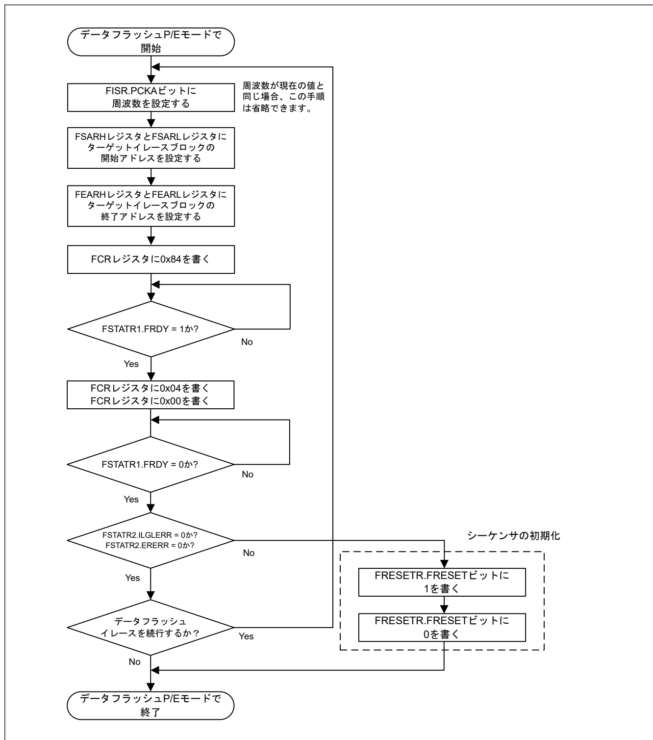
図 32.24 データフラッシュブロックイレース手順のフローチャート
