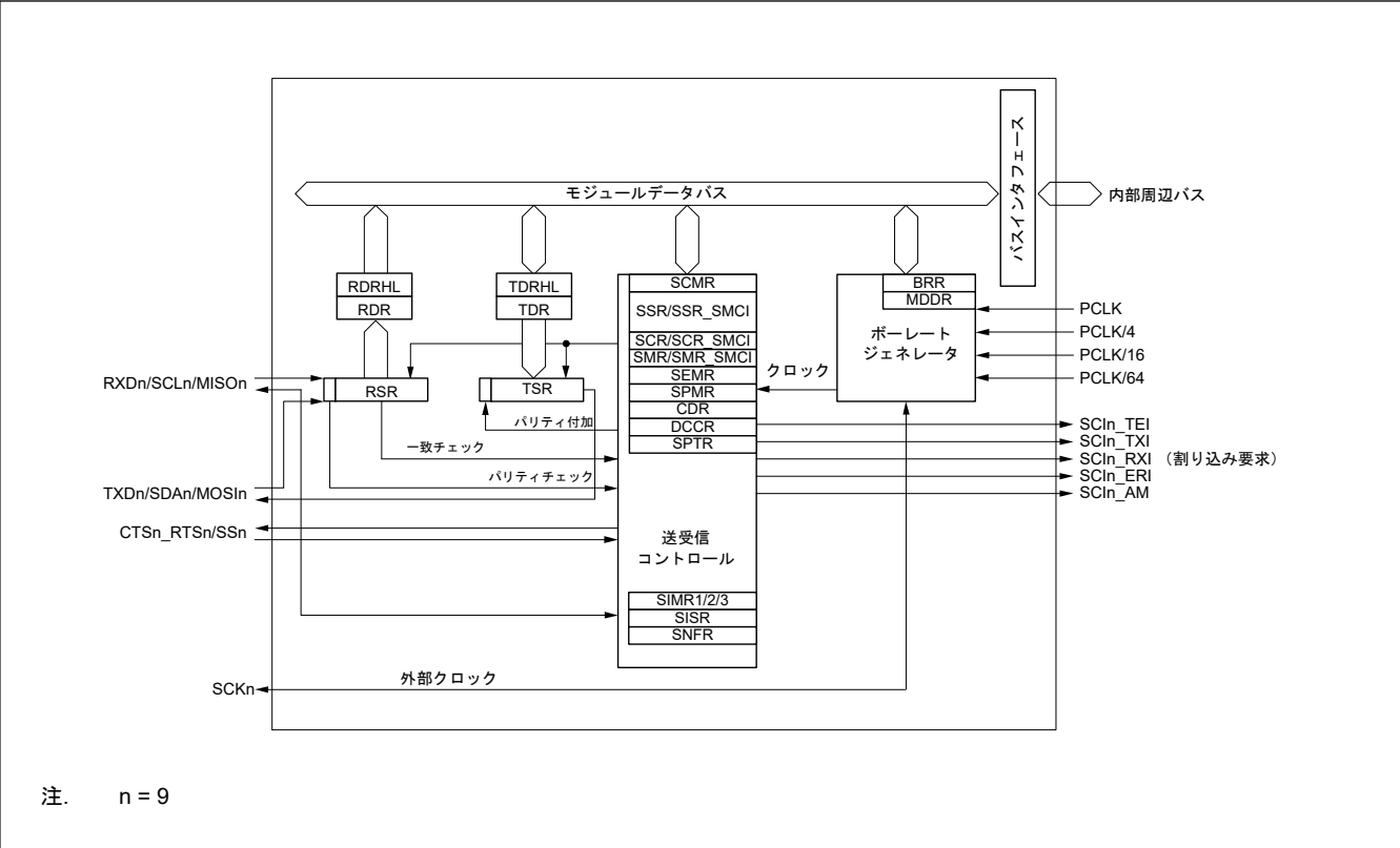
図 24.1 SCI のブロック図
