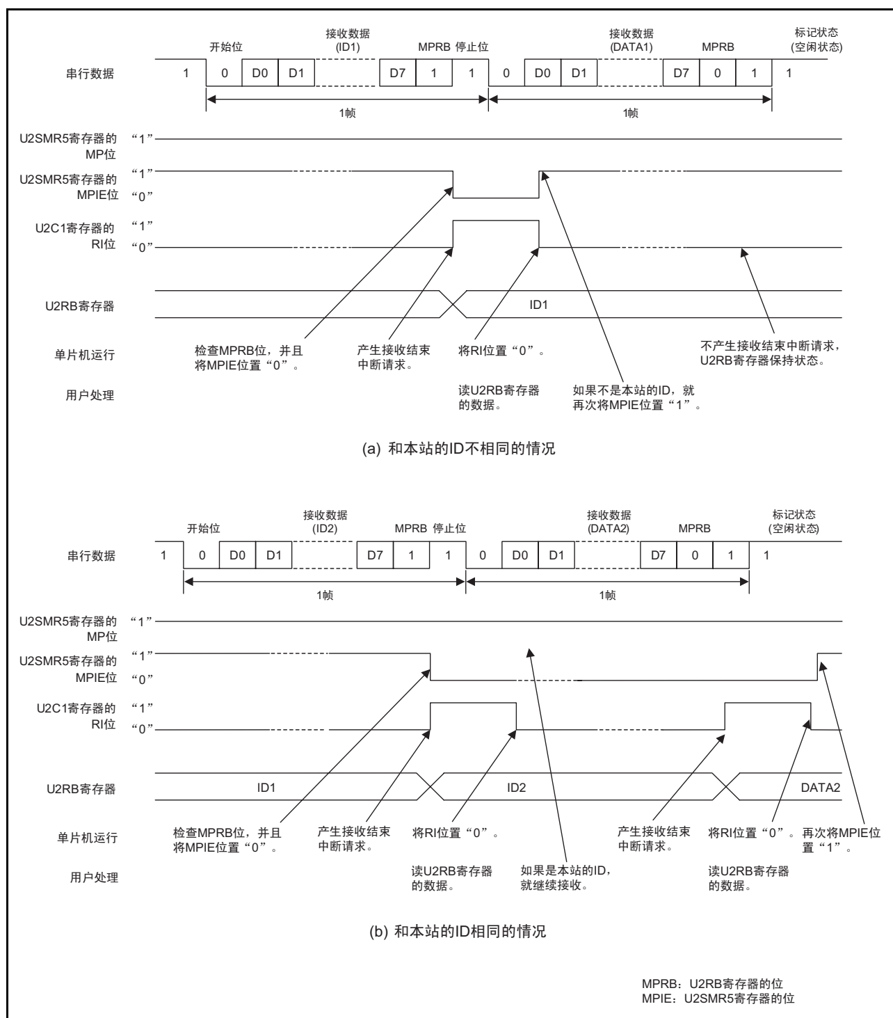
图 23.21 多处理器通信接收时的运行例子 (以 8 位数据 / 有多处理器位 / 1 位停止位为例)
