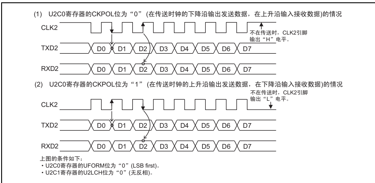
图 23.4 传送时钟的极性
