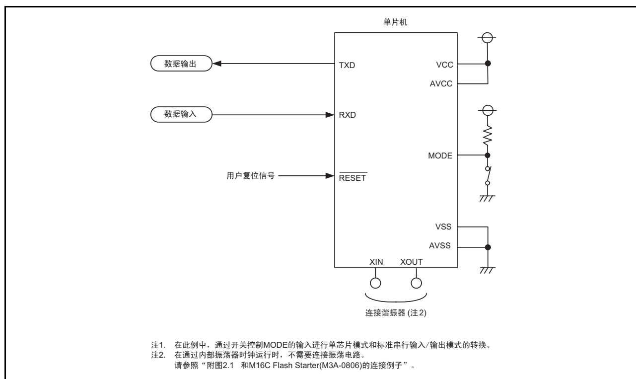
图 32.17 使用标准串行输入 / 输出模式 2 时的引脚处理例子
