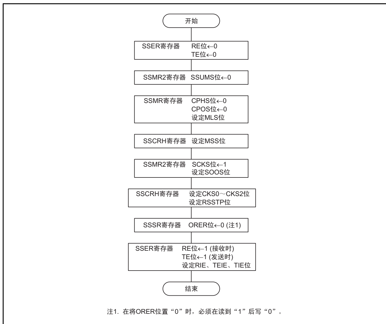
图 25.4 时钟同步通信模式的初始化
