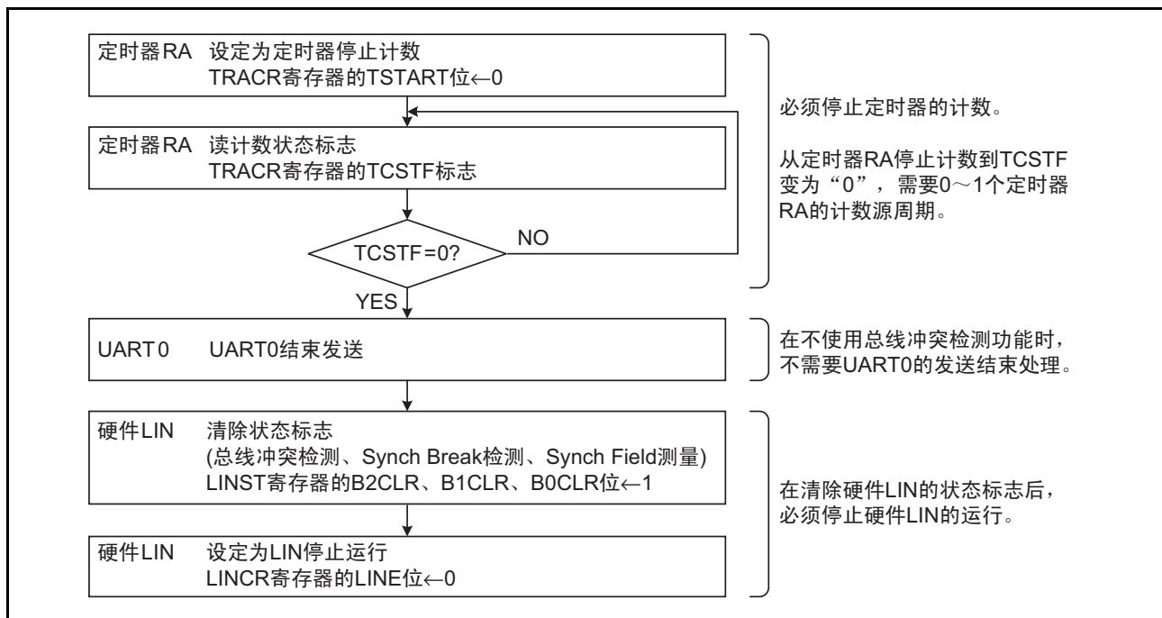
图 27.10 硬件 LIN 通信结束的流程图例子
