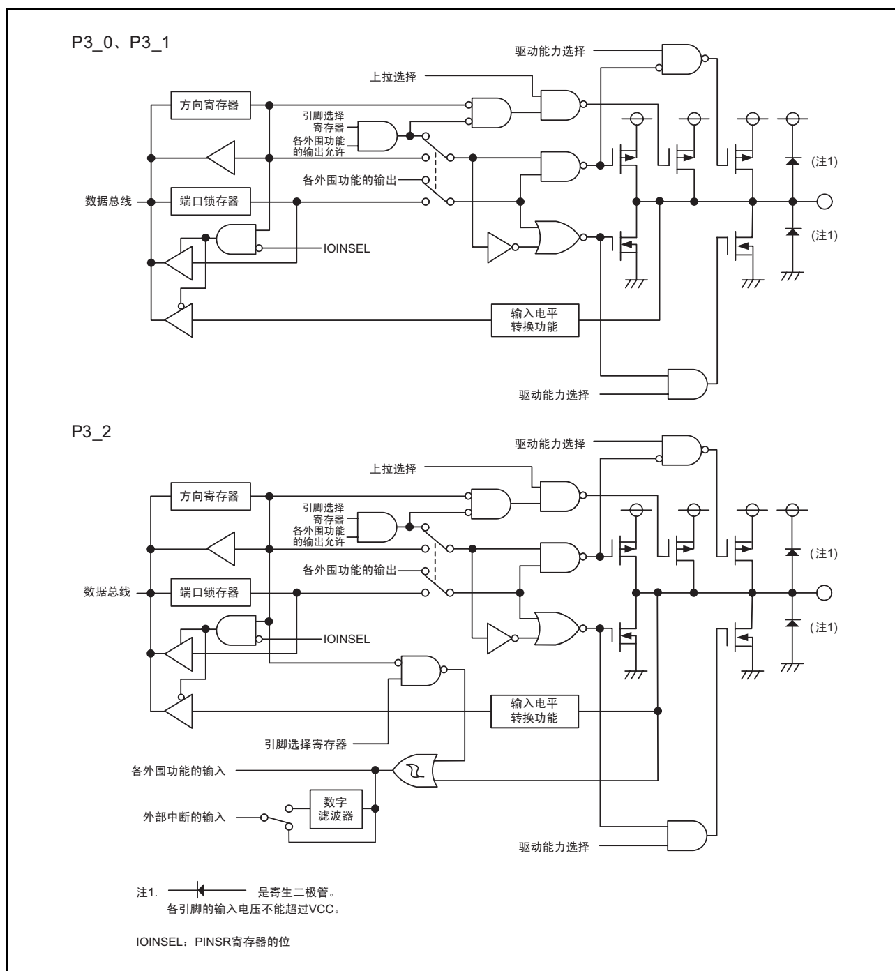
图 7.6 I/O 端口的结构 (6)
