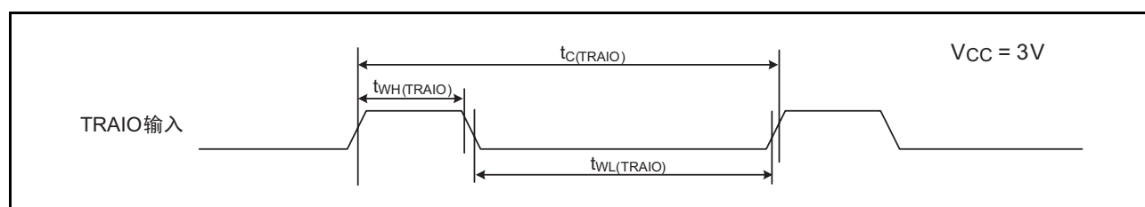
图 34.13 V_{CC}=3V 时的 TRAIO 输入时序
