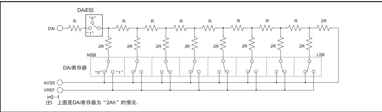
图 29.2 D/A 转换器的等效电路
