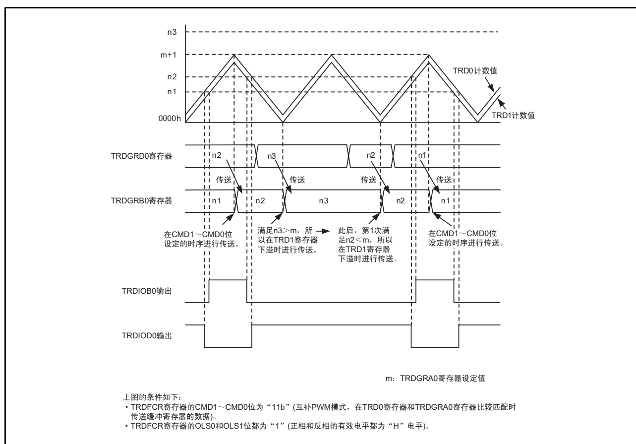
图 20.27 互补 PWM 模式中的缓冲寄存器的值 \geq TRDGRA0 寄存器的值时的运行例子
