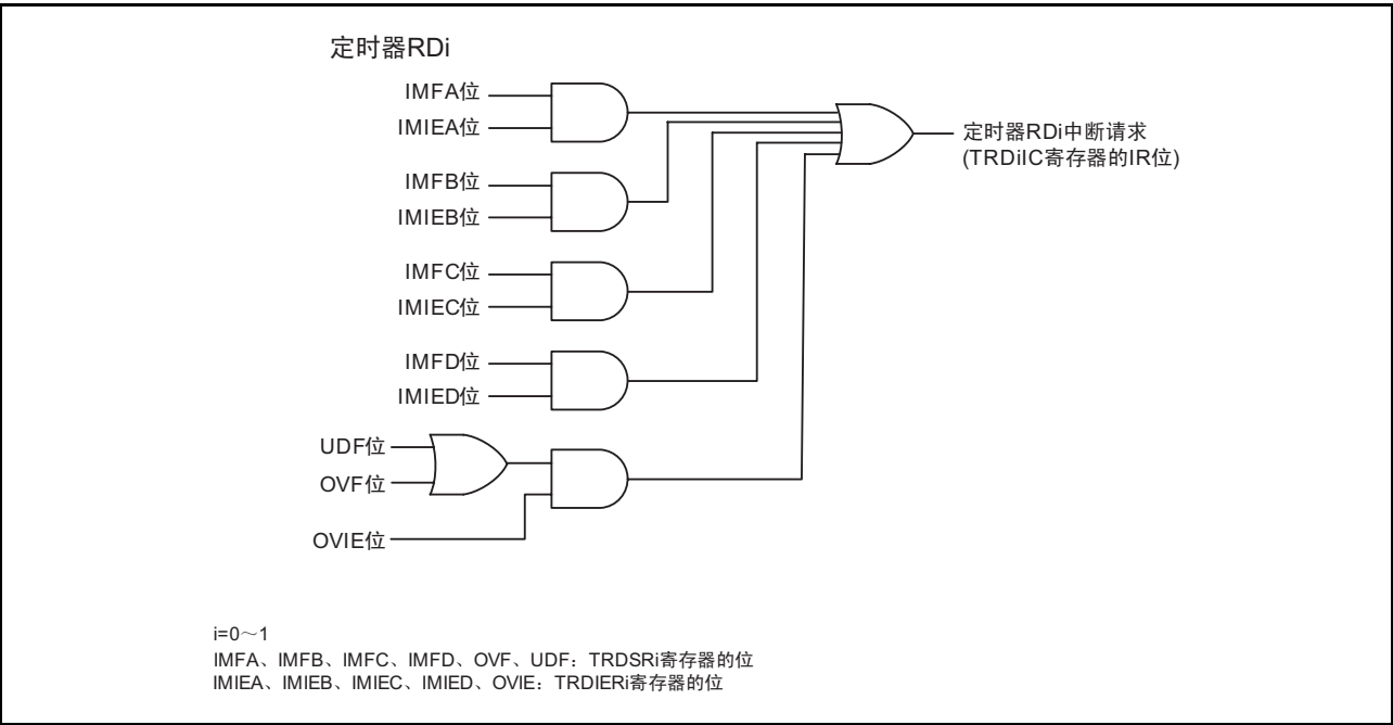
图 11.12 定时器 RD 中断的框图
