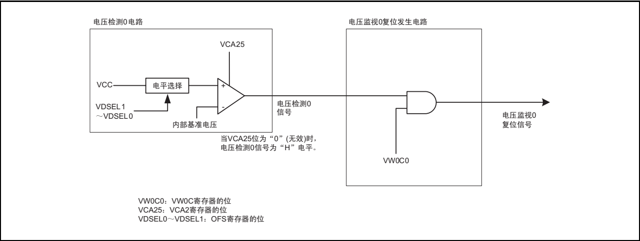
图 6.2 电压监视 0 复位发生电路的框图
