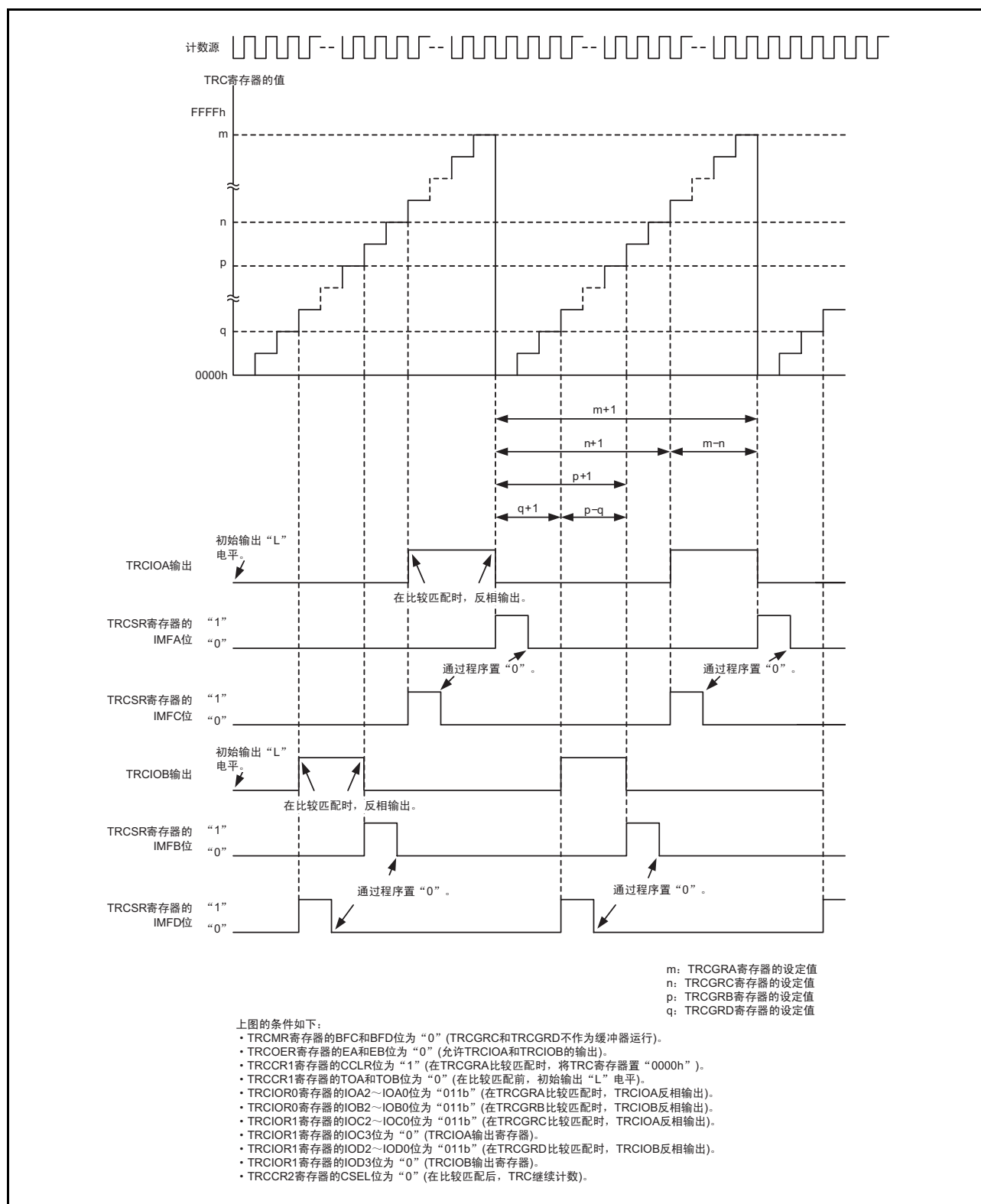
图 19.12 将 TRCGRC 和 TRCGRD 分别用于 TRCIOA 引脚和 TRCIOB 引脚的输出控制时的运行例子
