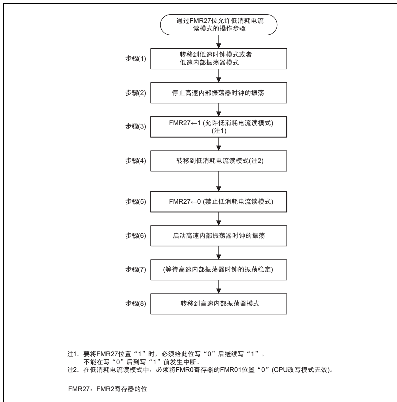
图 33.3 低消耗电流读模式的操作步骤例子
