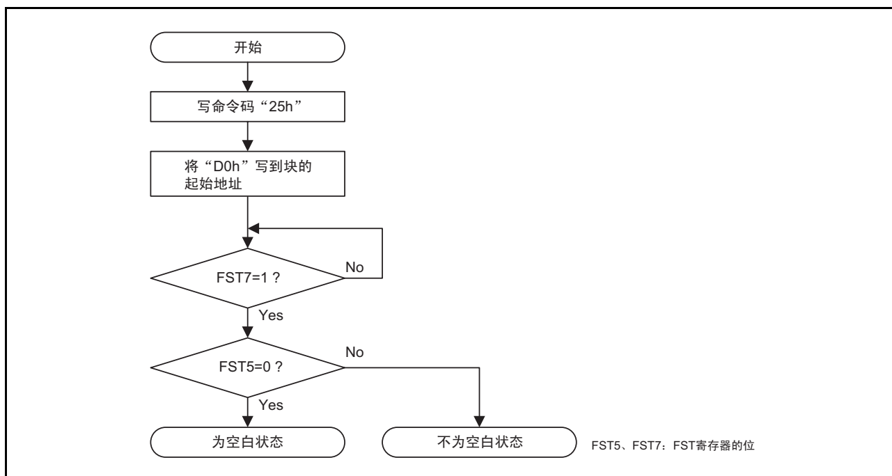
图 32.15 块空白检查的流程图
