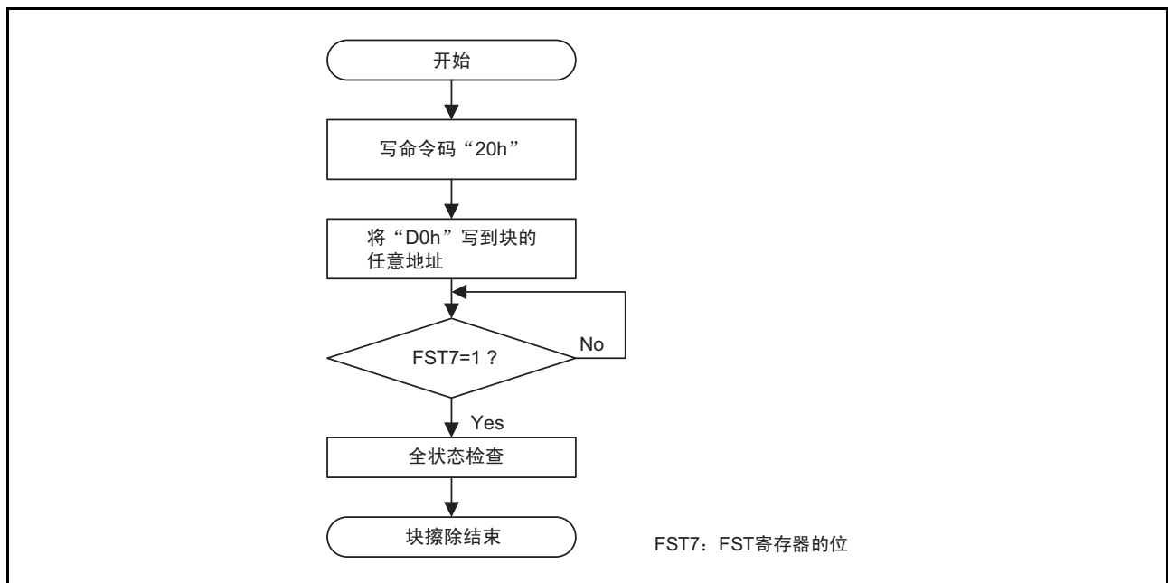
图 32.10 块擦除的流程图（禁止闪存就绪状态的中断）
