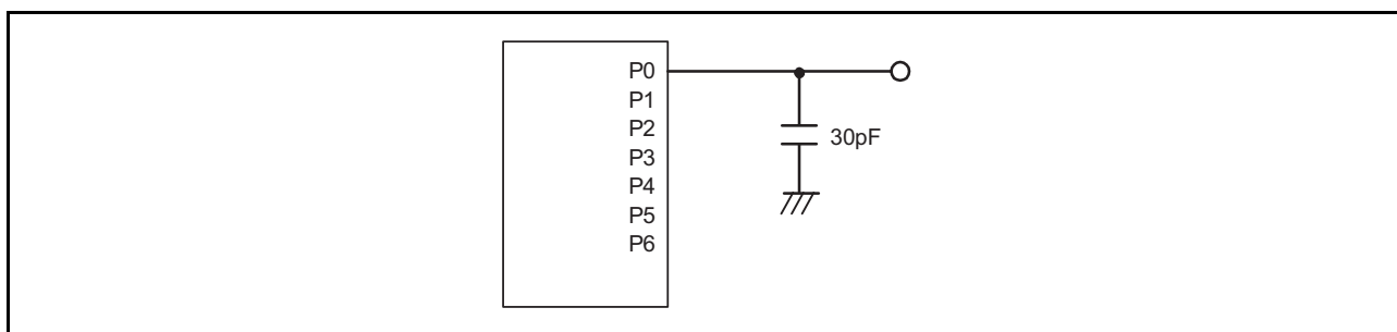
图 34.1 端口 P0 ~ P6 的时序测量电路
