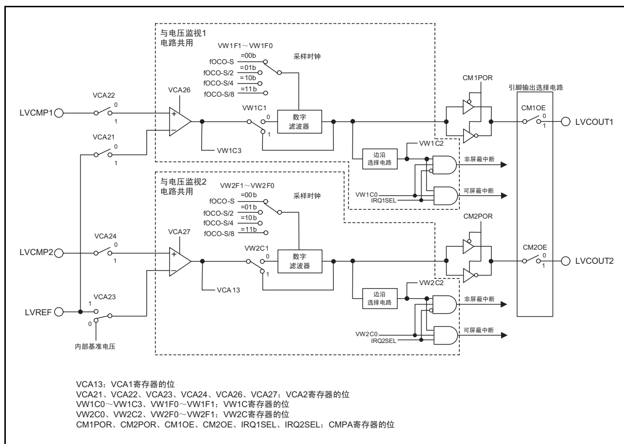
图 30.1 比较电路 A 的框图
