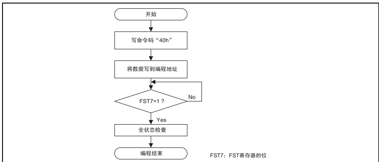
图 32.8 编程的流程图（禁止闪存就绪状态的中断）
