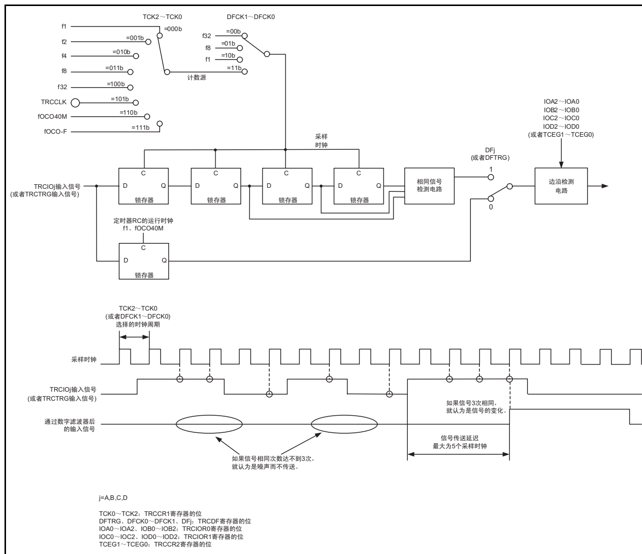
图 19.5 数字滤波器的框图
