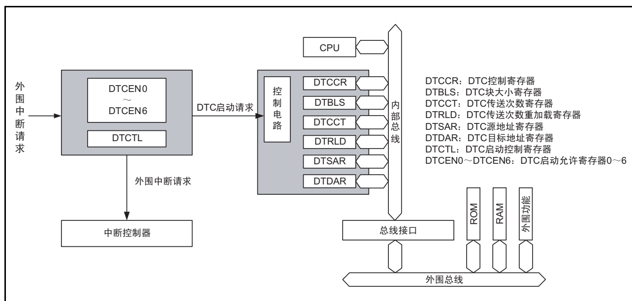
图 15.1 DTC 的框图
