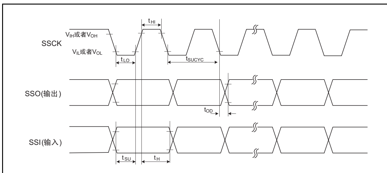
图 34.6 带片选的时钟同步串行 I/O 的输入 / 输出时序（时钟同步通信模式）
