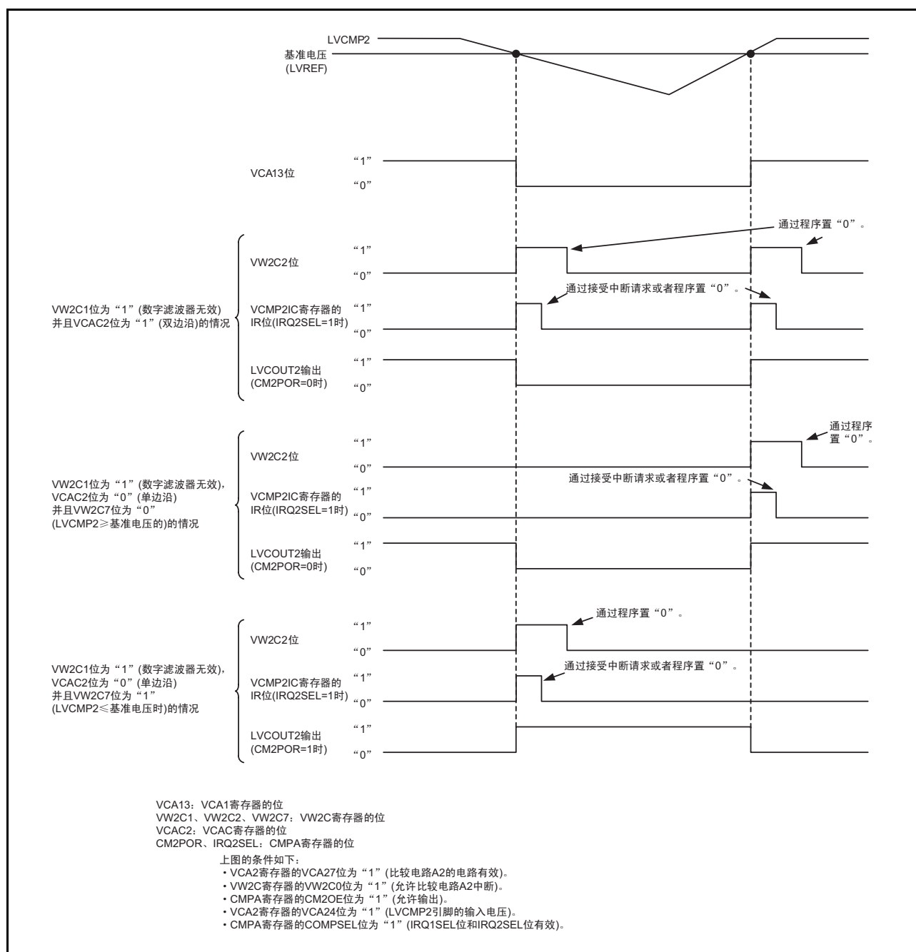
图 30.5 比较电路 A2 的运行例子 (数字滤波器无效)
