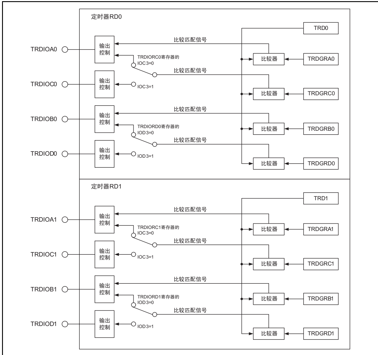
图 20.12 TRDGRCi 和 TRDGRDi 的输出引脚的变更
