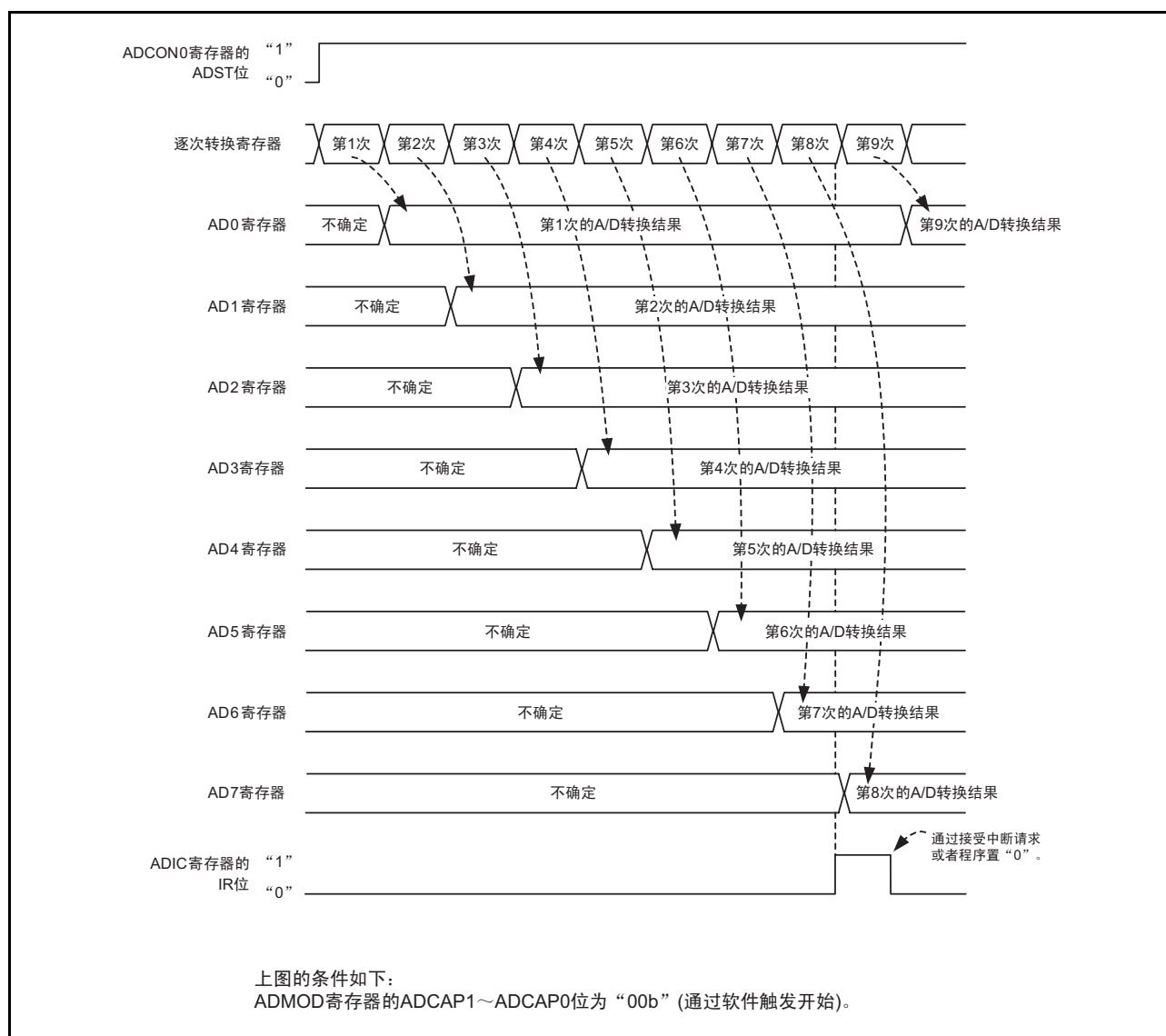
图 28.7 重复模式 1 的运行例子
