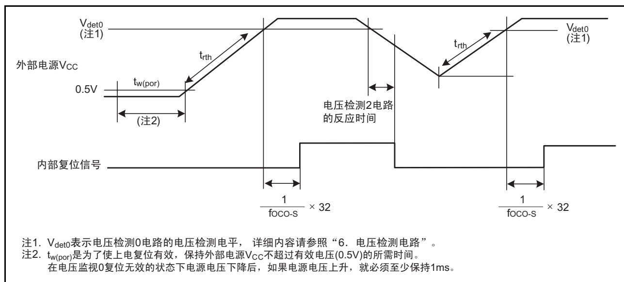
图 34.3 上电复位电路的电特性
