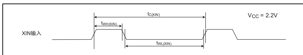
图 34.16 V_{CC}=2.2V 时的 XIN 和 XCIN 的输入时序
