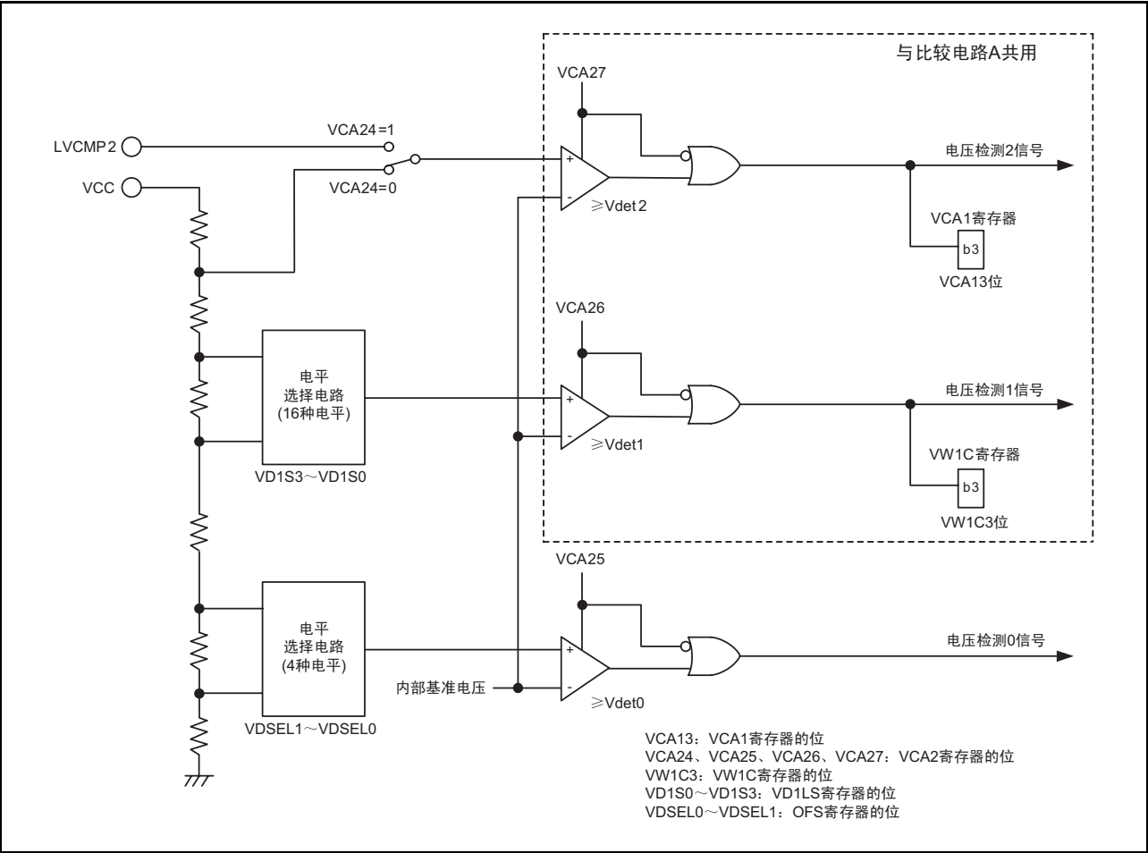
图 6.1 电压检测电路的框图
