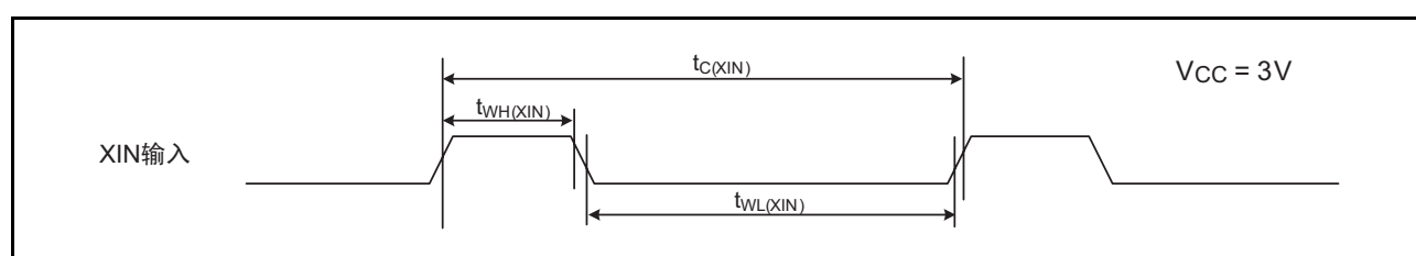
图 34.12 V_{CC}=3V 时的 XIN 和 XCIN 的输入时序
