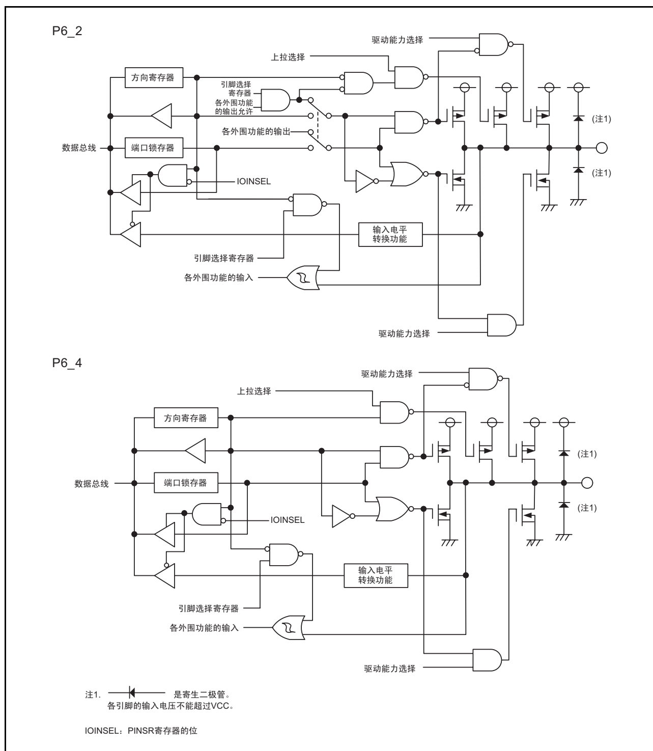
图 7.15 I/O 端口的结构 (15)
