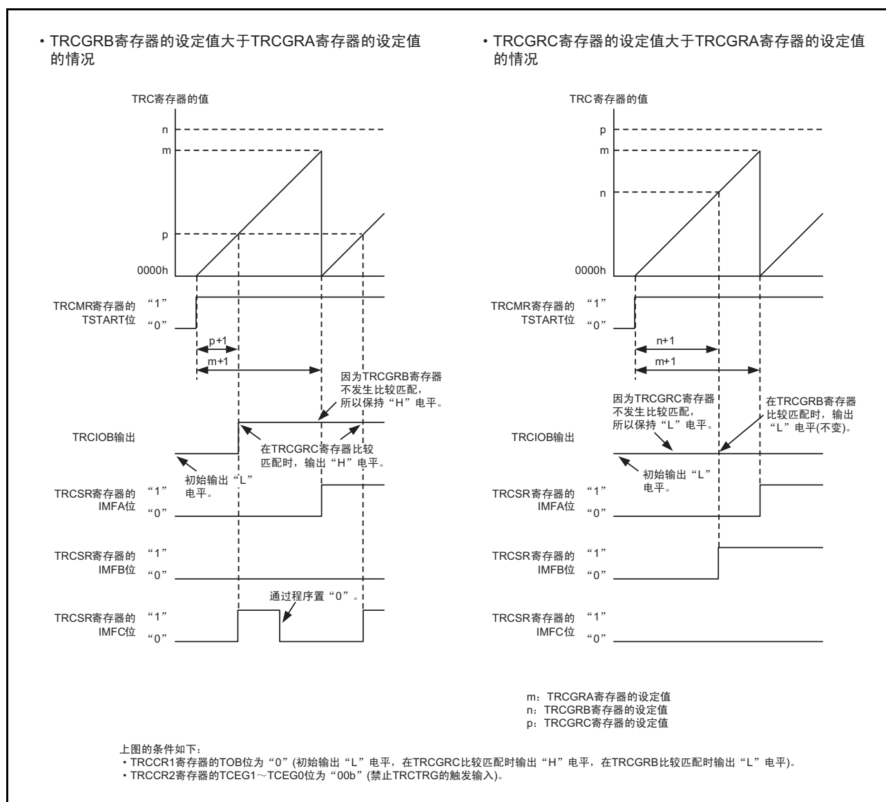
图 19.19 PWM2 模式的运行例子（占空比为 0% 和 100%）
