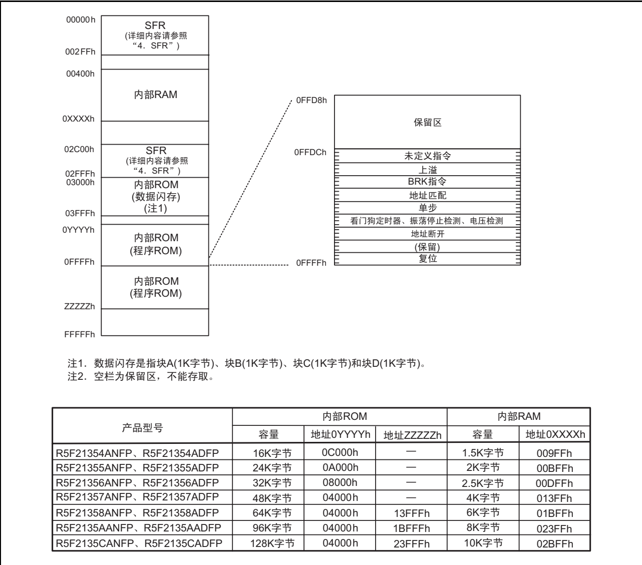
图 3.1 R8C/35A 群的存储器分配图
