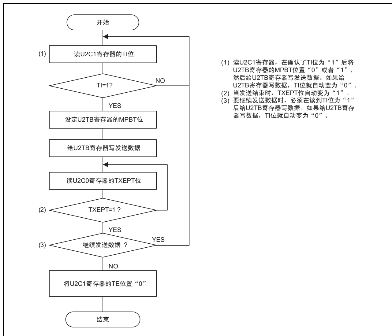
图 23.19 多处理器数据发送的流程图例子
