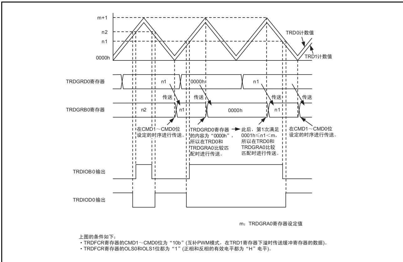
图 35.5 互补 PWM 模式中的缓冲寄存器的值为“0000h”时的运行例子
