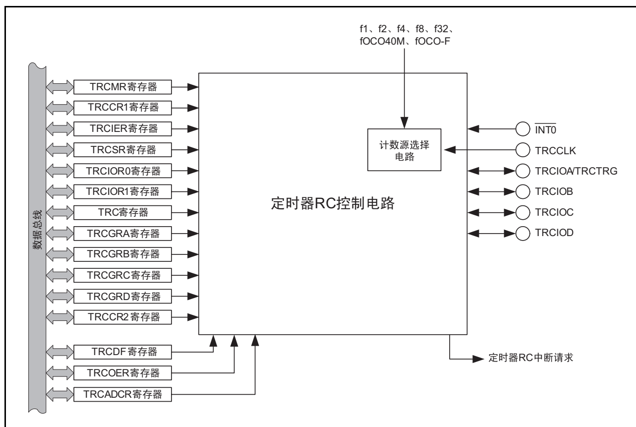
图 19.1 定时器 RC 的框图
