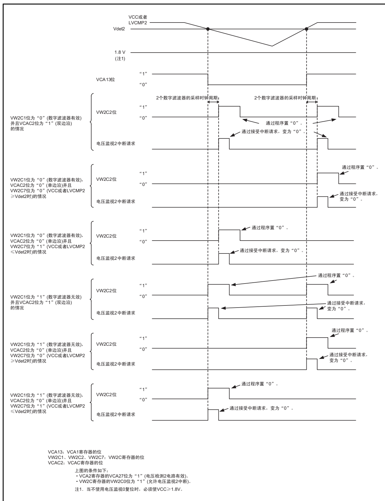
图 6.7 电压监视 2 中断的运行例子
