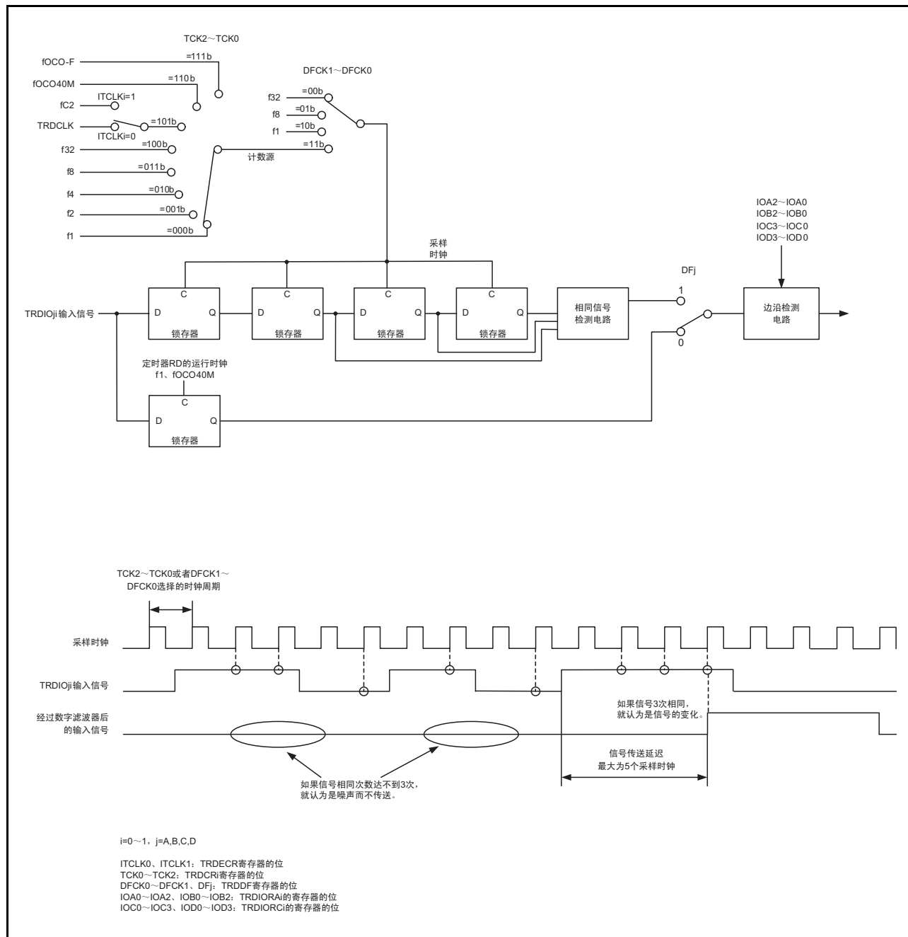
图 20.9 数字滤波器的框图
