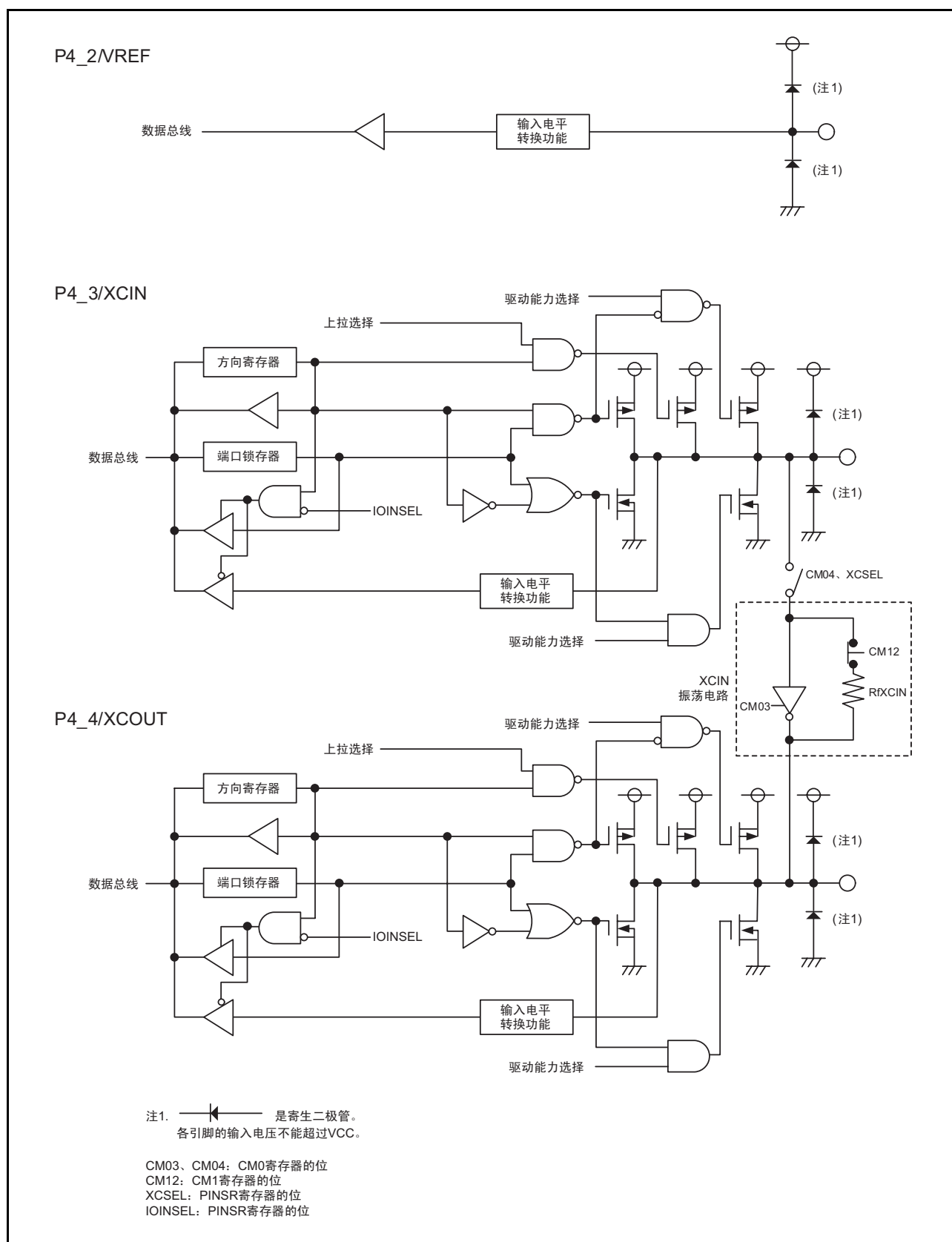
图 7.10 I/O 端口的结构 (10)
