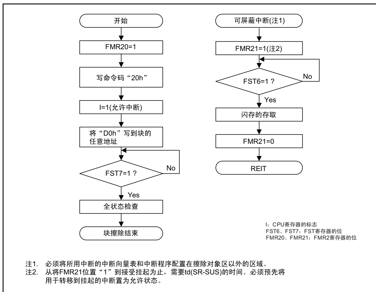
图 32.11 块擦除的流程图（禁止闪存就绪状态的中断而允许挂起）
