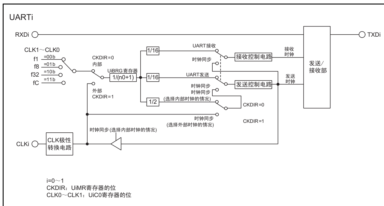
图 22.1 UARTi (i=0 ~ 1) 的框图
