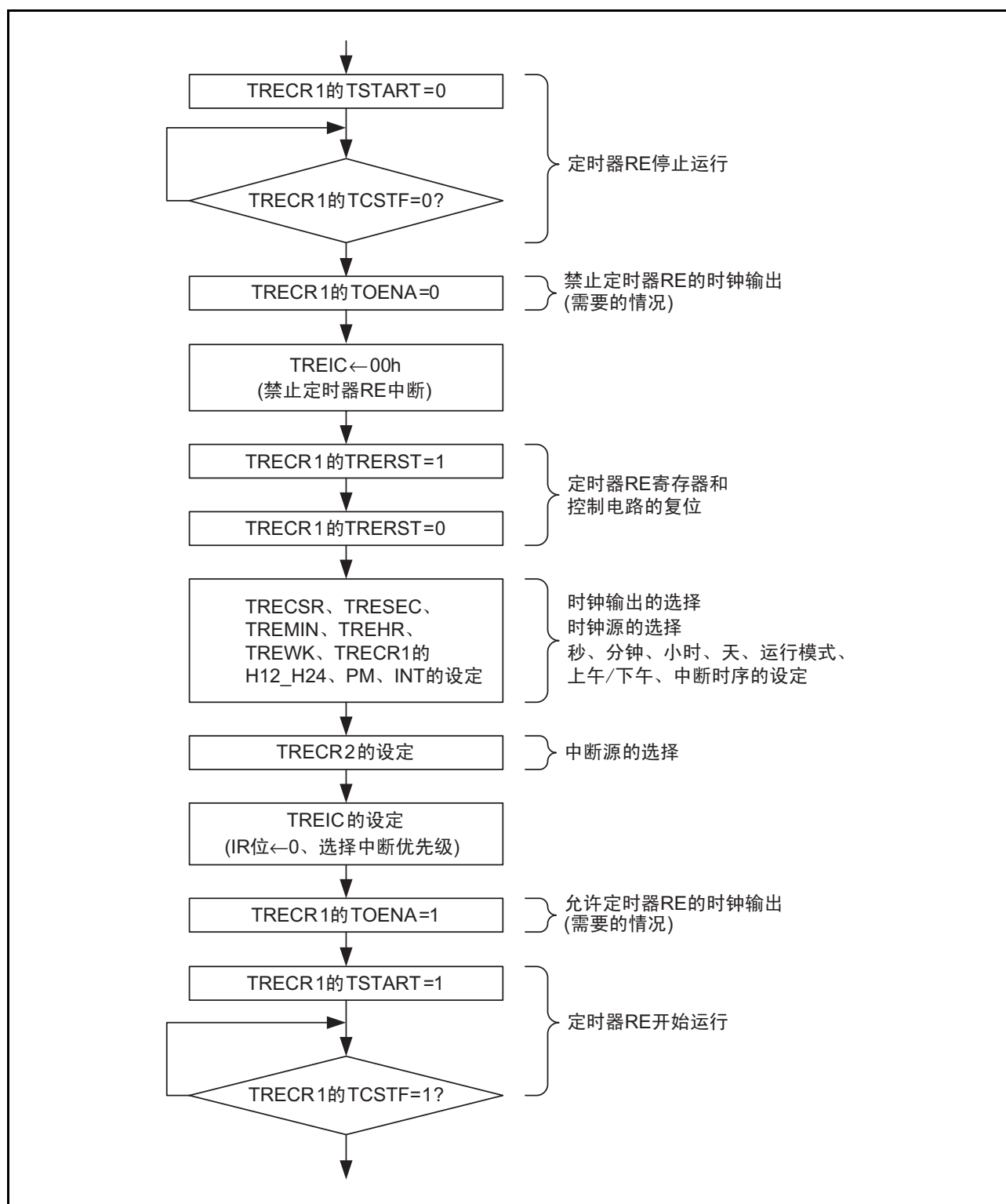
图 35.6 实时时钟模式的设定例子
