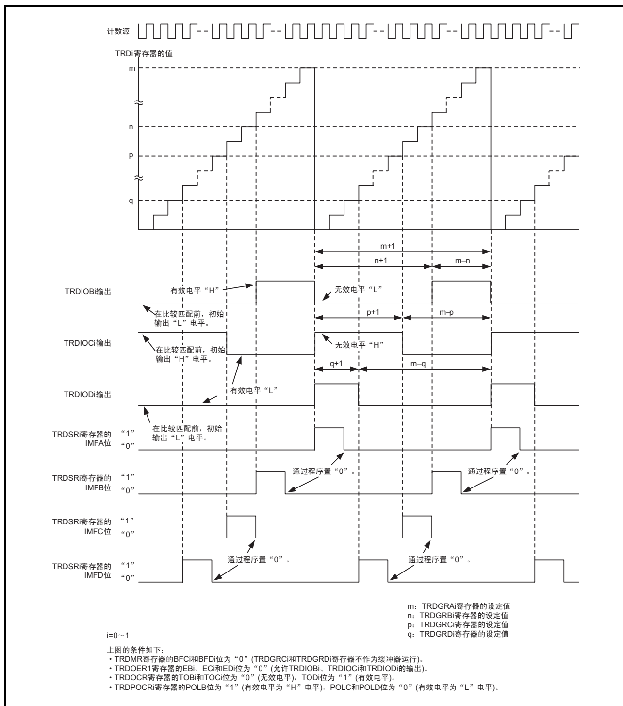
图 20.15 PWM 模式的运行例子
