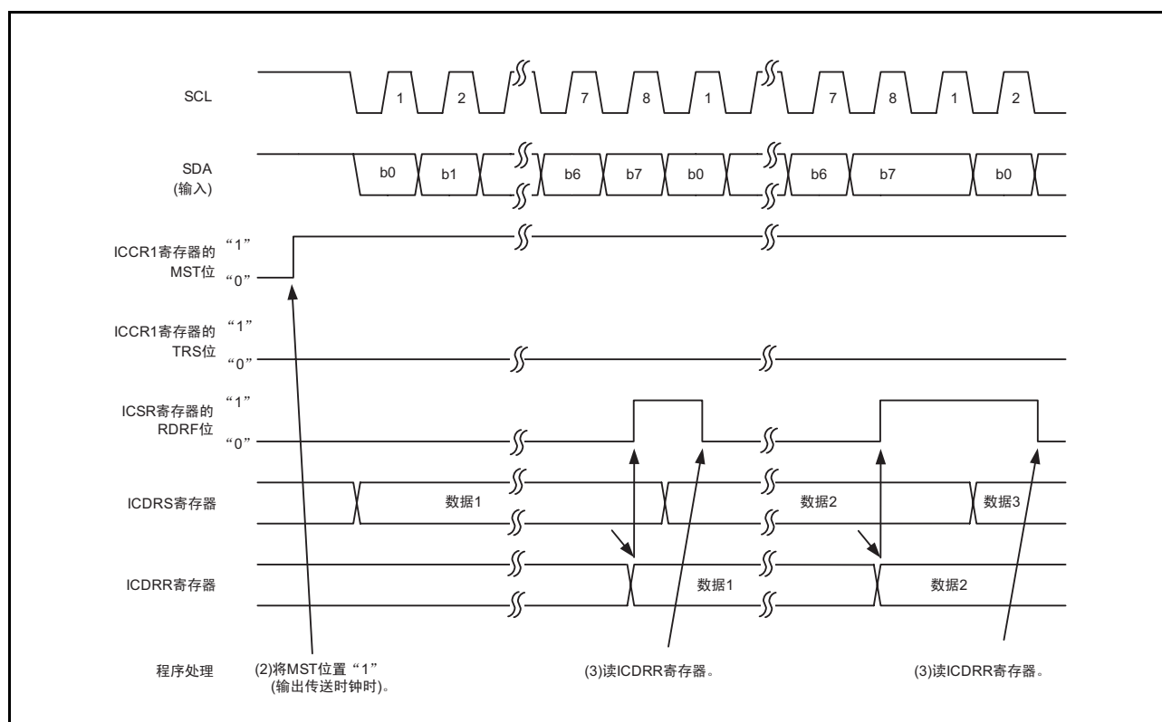
图 26.15 接收模式的运行时序（时钟同步串行模式）
