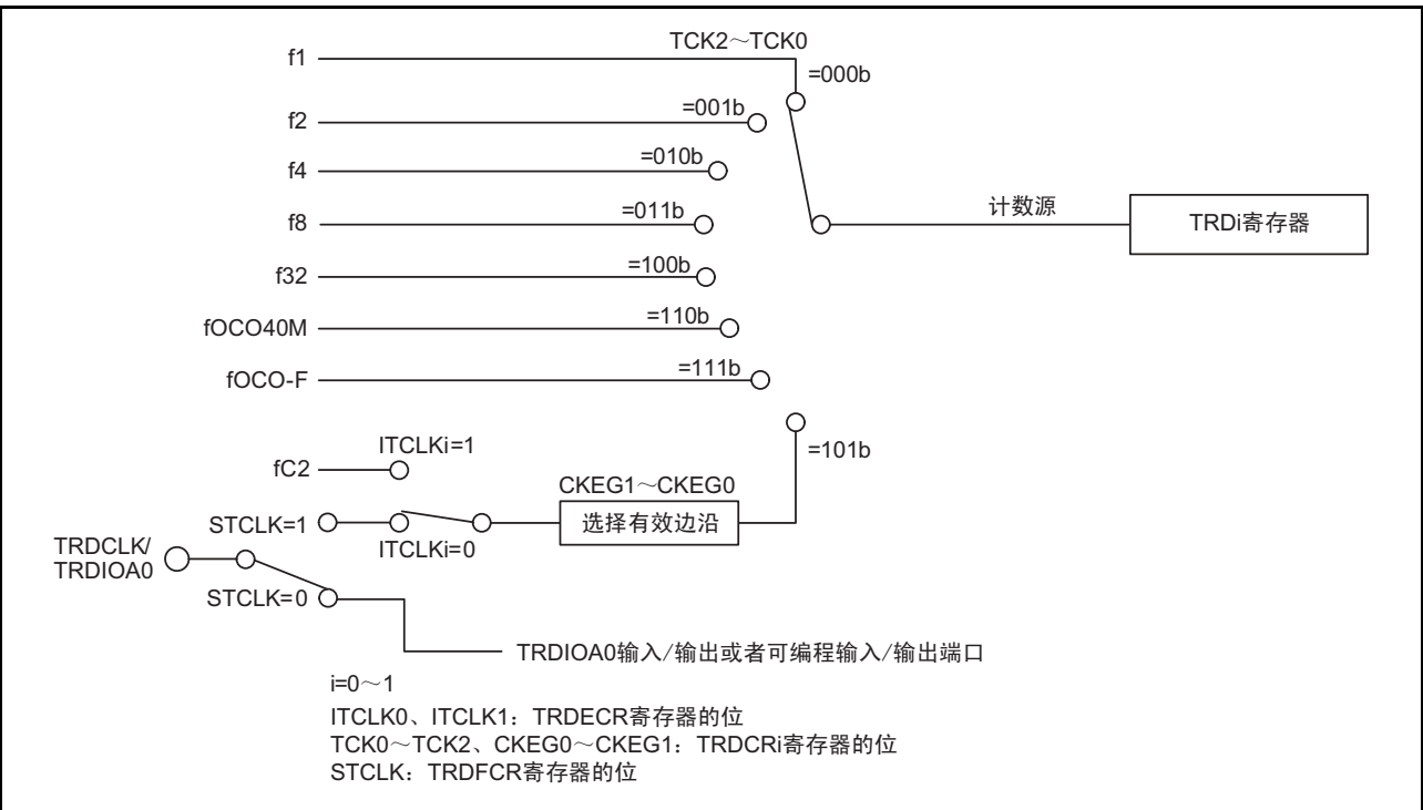
图 20.2 计数源的框图
