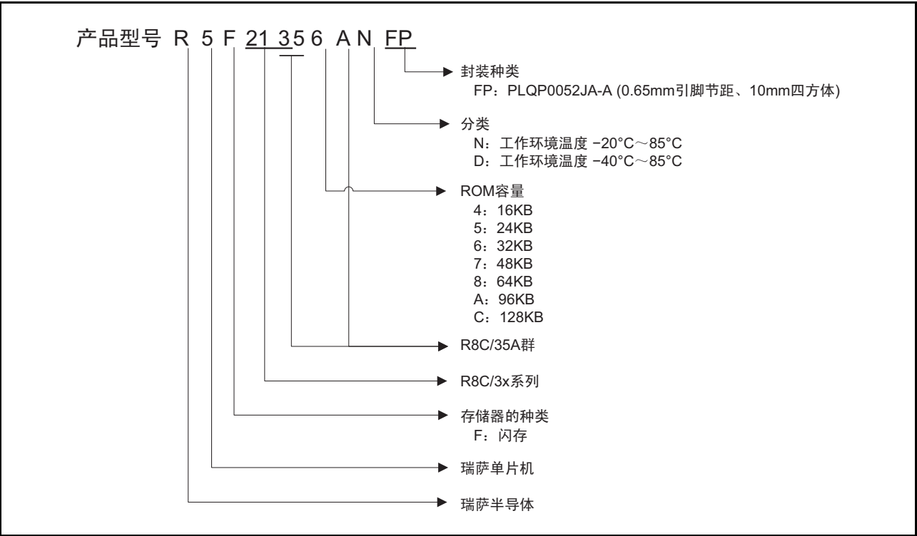
图 1.1 R8C/35A 群的产品型号、存储器容量和封装
