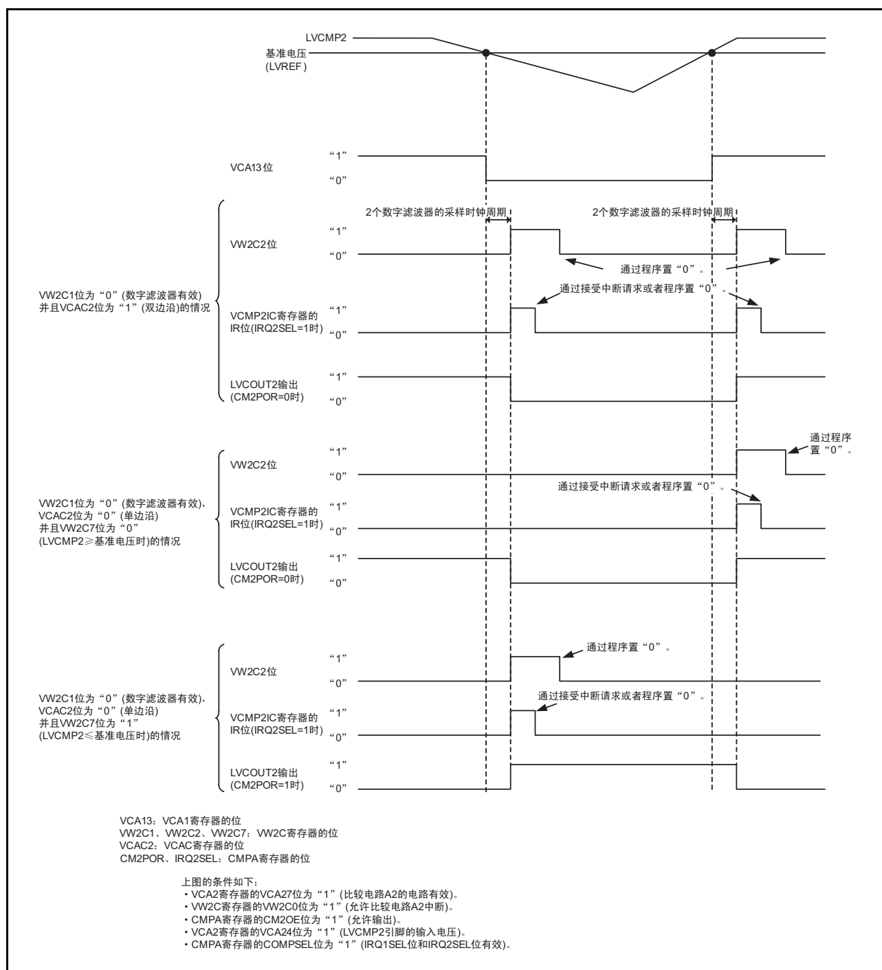
图 30.4 比较电路 A2 的运行例子（数字滤波器有效）
