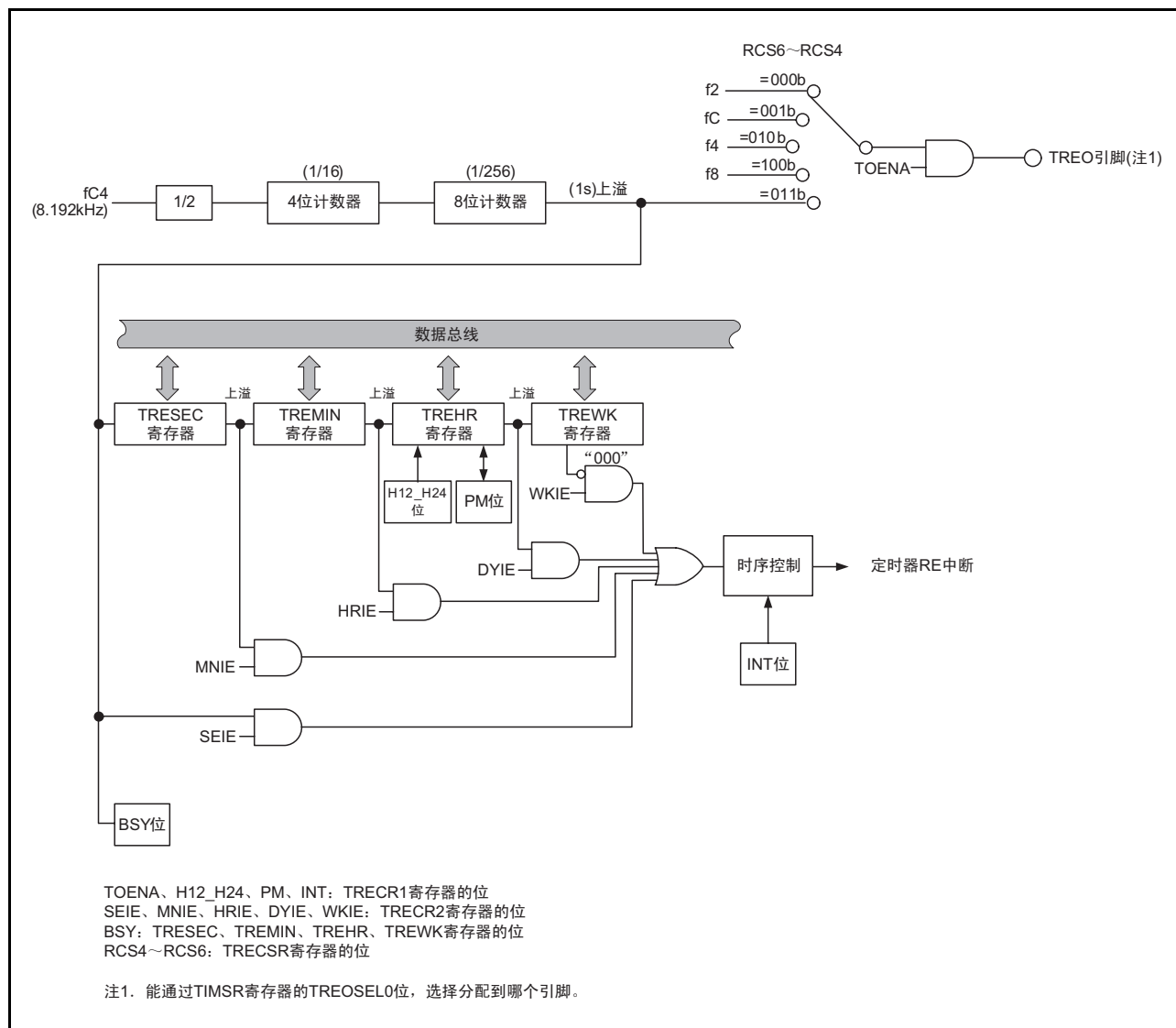
图 21.1 实时时钟模式的框图
