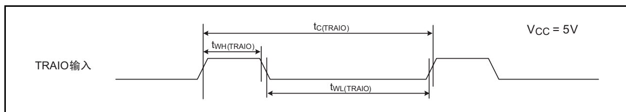
图 34.9 V_{CC}=5V 时的 TRAIO 输入时序
