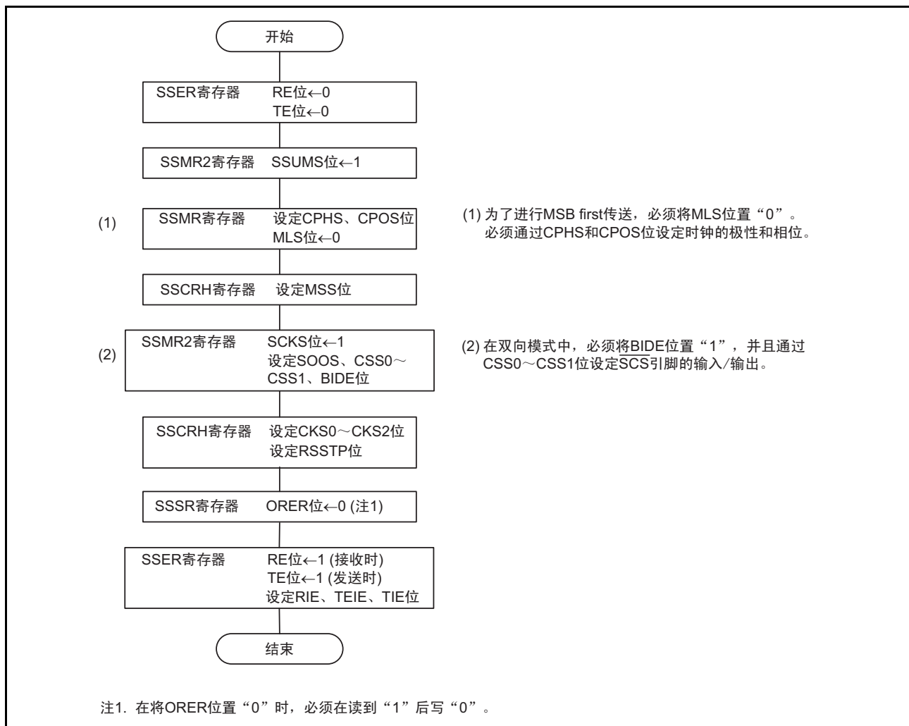
图 25.10 4 线式总线通信模式的初始化
