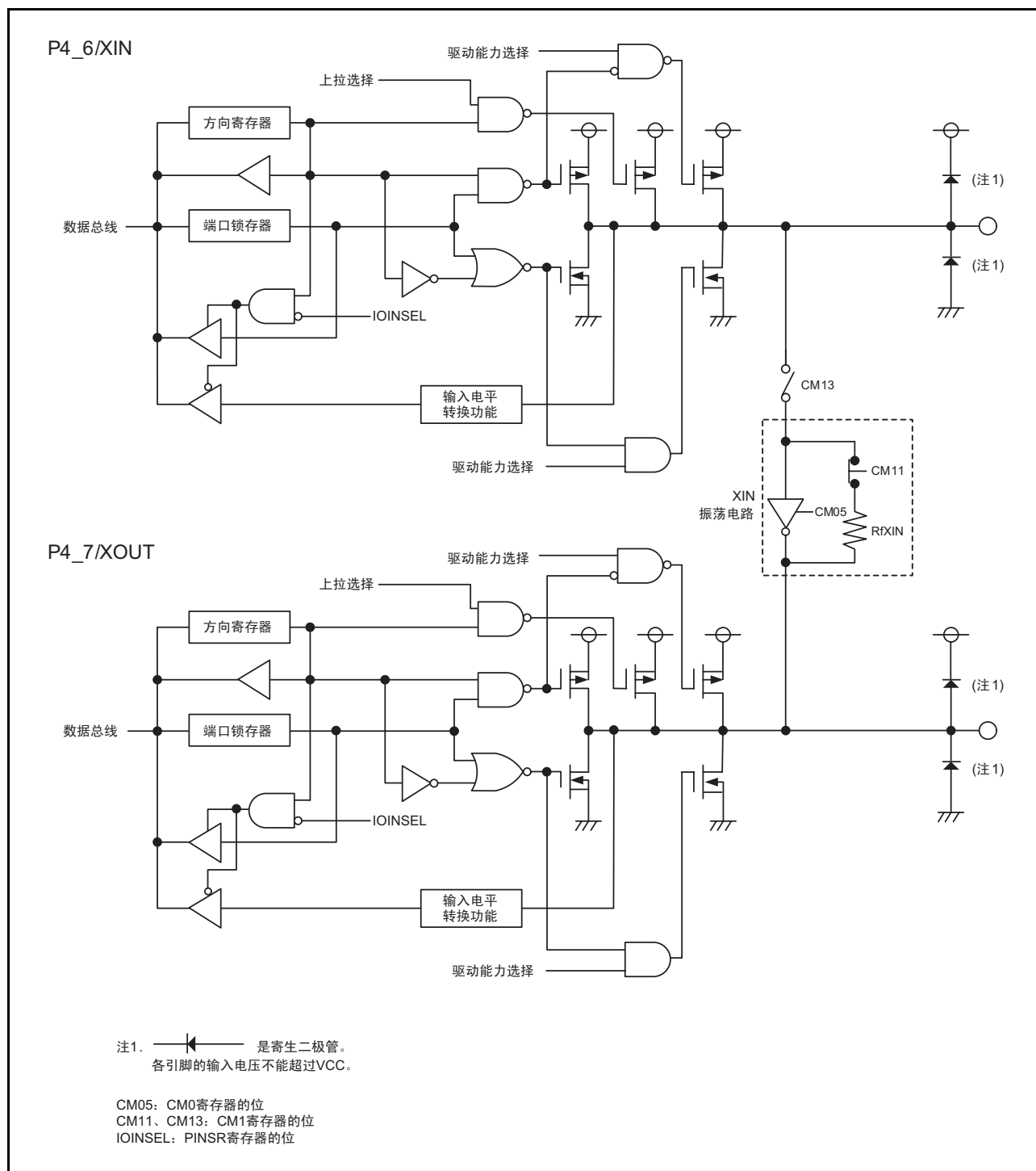
图 7.12 I/O 端口的结构 (12)
