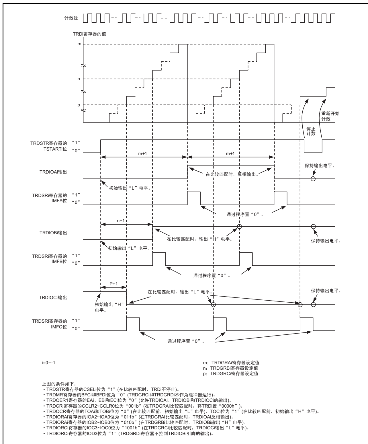
图 20.11 输出比较功能的运行例子
