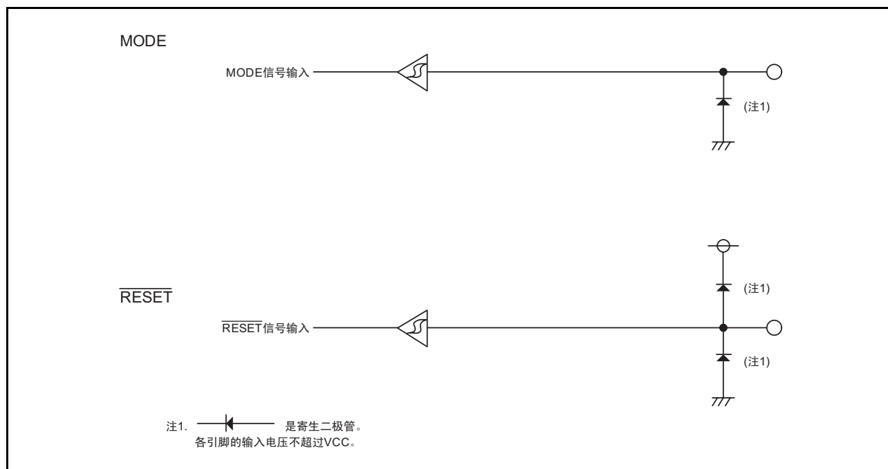
图 7.17 引脚的结构
