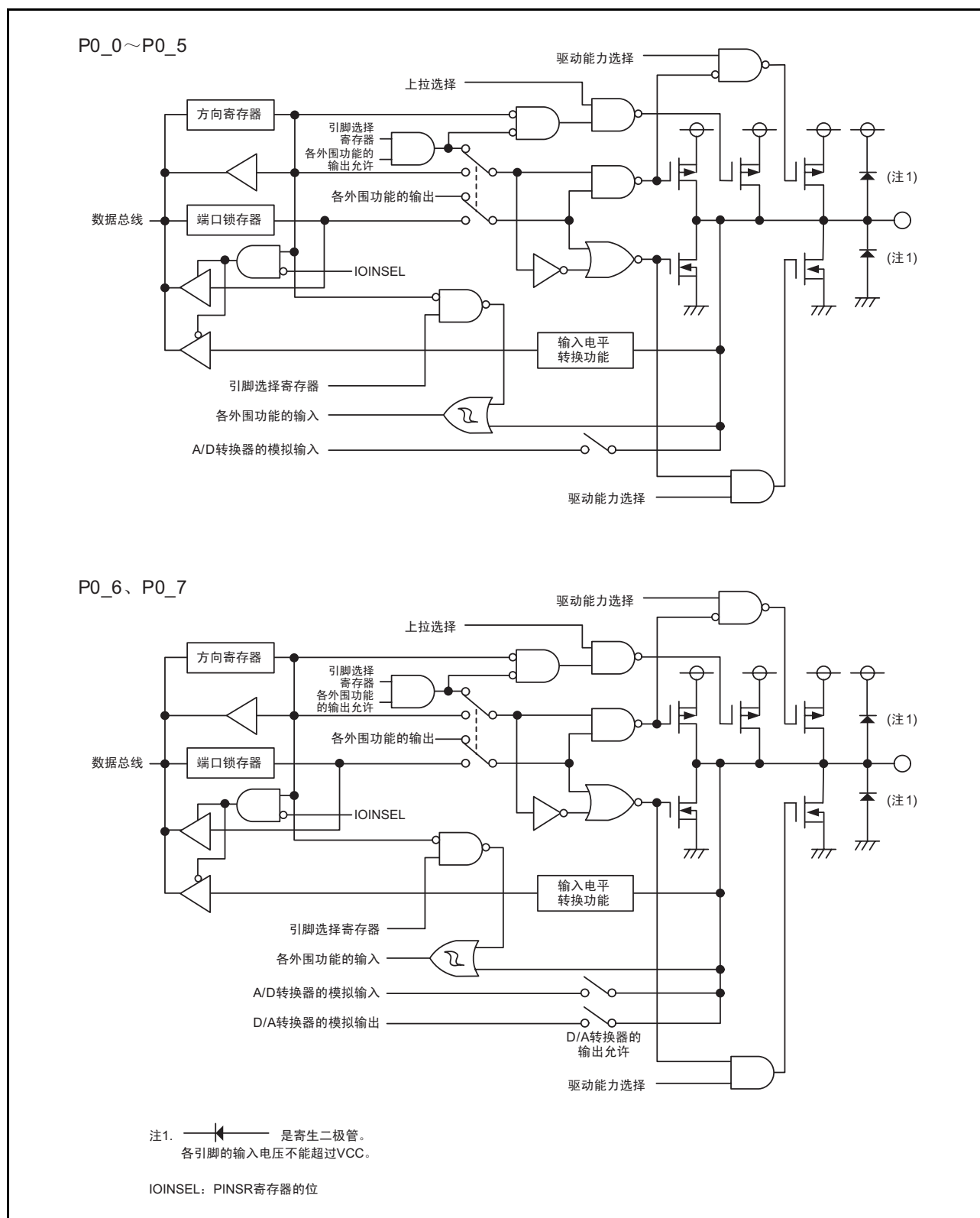
图 7.1 I/O 端口的结构 (1)
