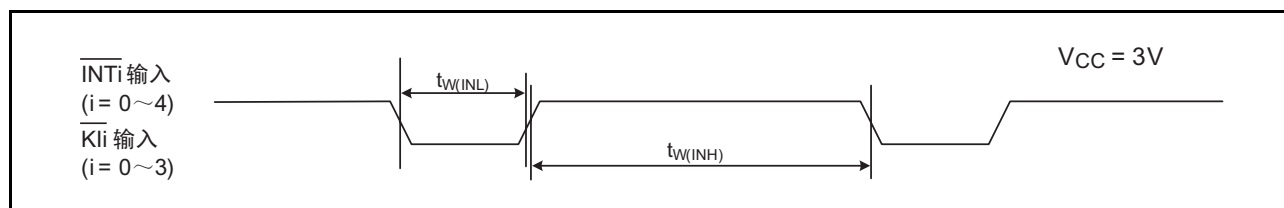
图 34.15 V_{CC}=3V 时的外部中断 \overline{INTi} 和键输入中断 \overline{Kli} 的输入时序
