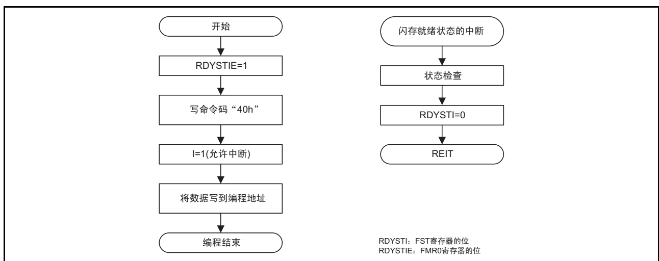
图 32.9 编程的流程图（允许闪存就绪状态的中断）
