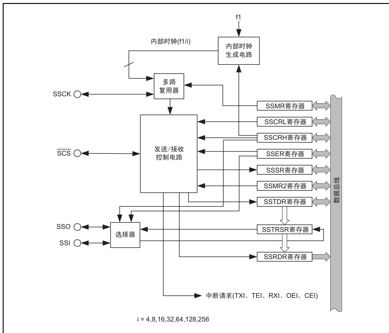
图 25.1 同步串行通信单元的框图
