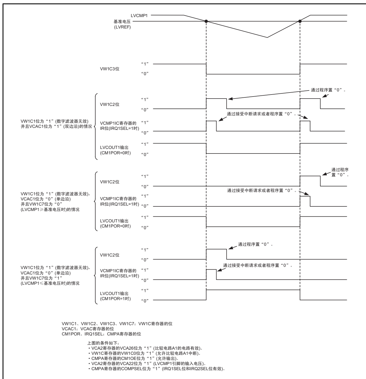
图 30.3 比较电路 A1 的运行例子 (数字滤波器无效)
