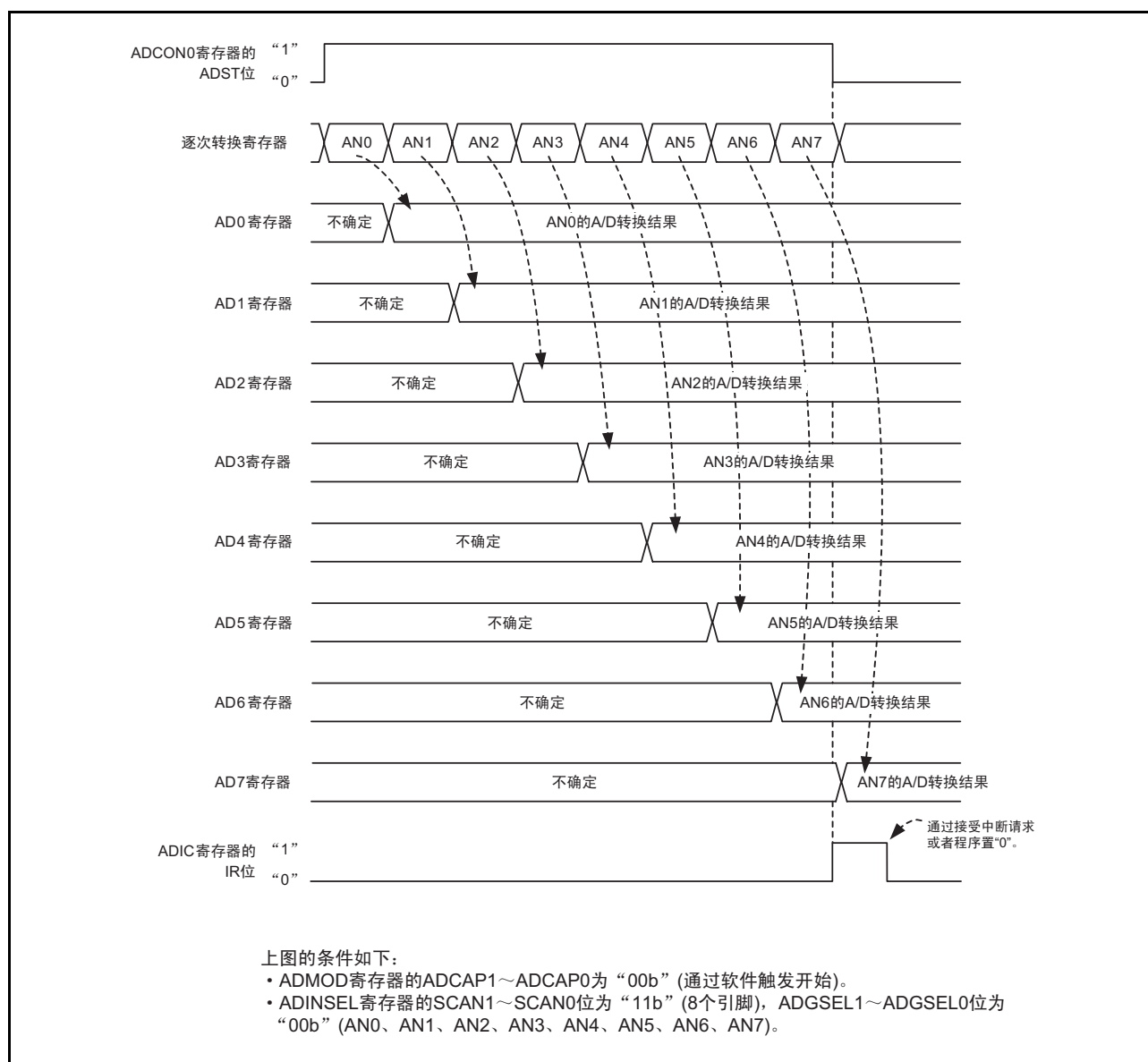
图 28.8 单次扫描模式的运行例子
