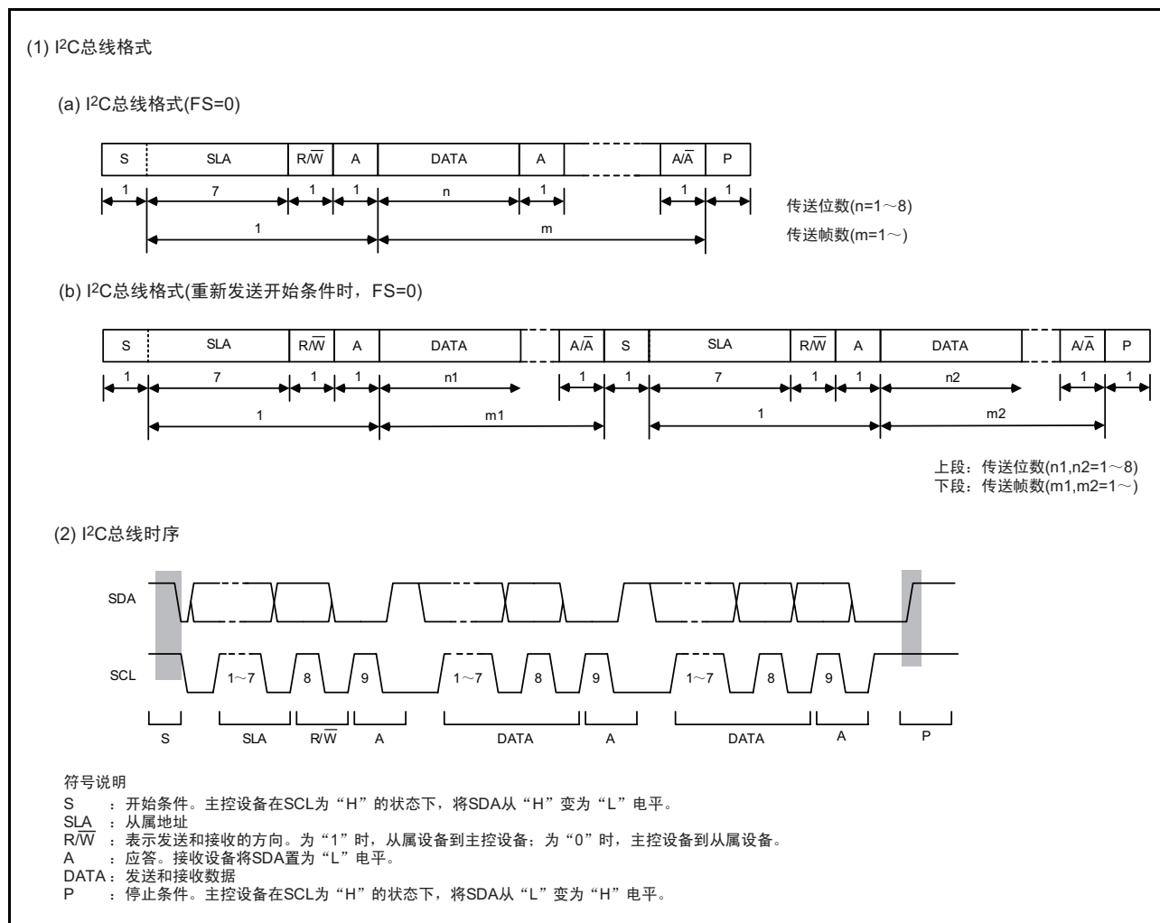
图 26.4 I 2 C 总线格式和总线时序
