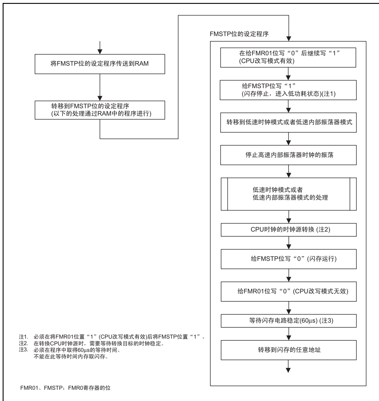
图 33.2 通过 FMSTP 位降低功耗的操作步骤例子
