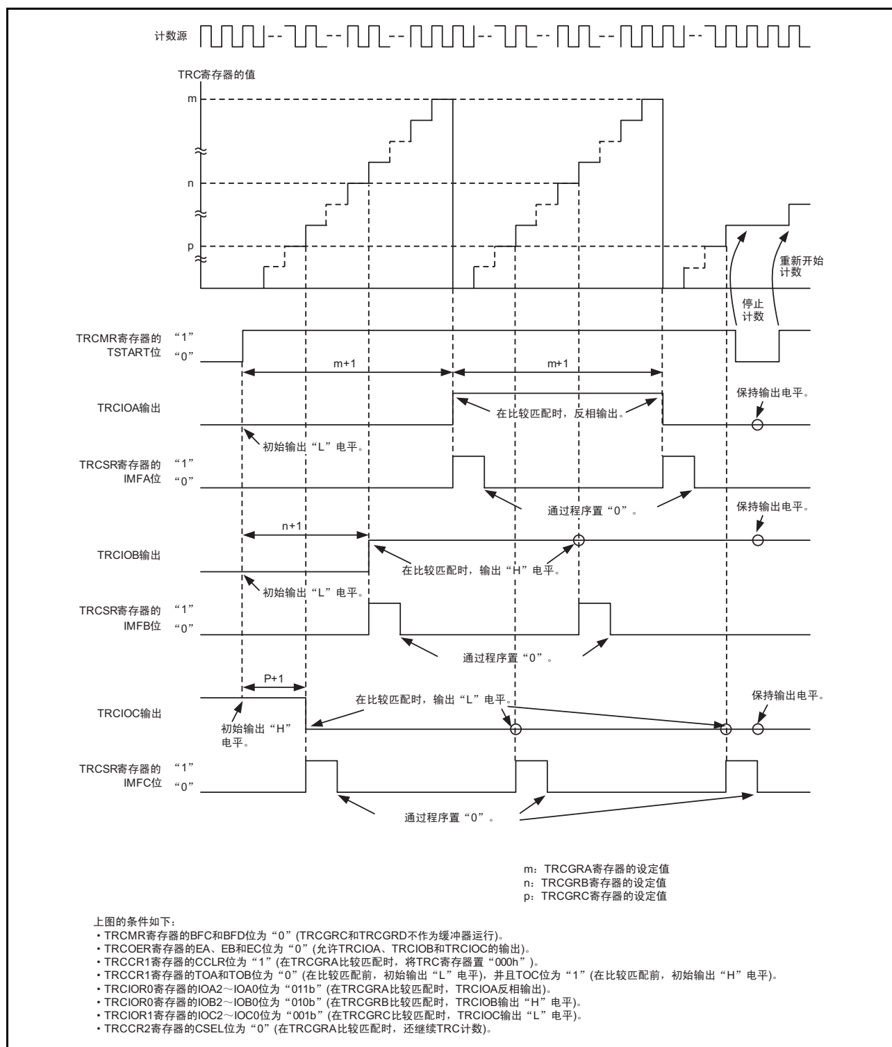
图 19.10 输出比较功能的运行例子
