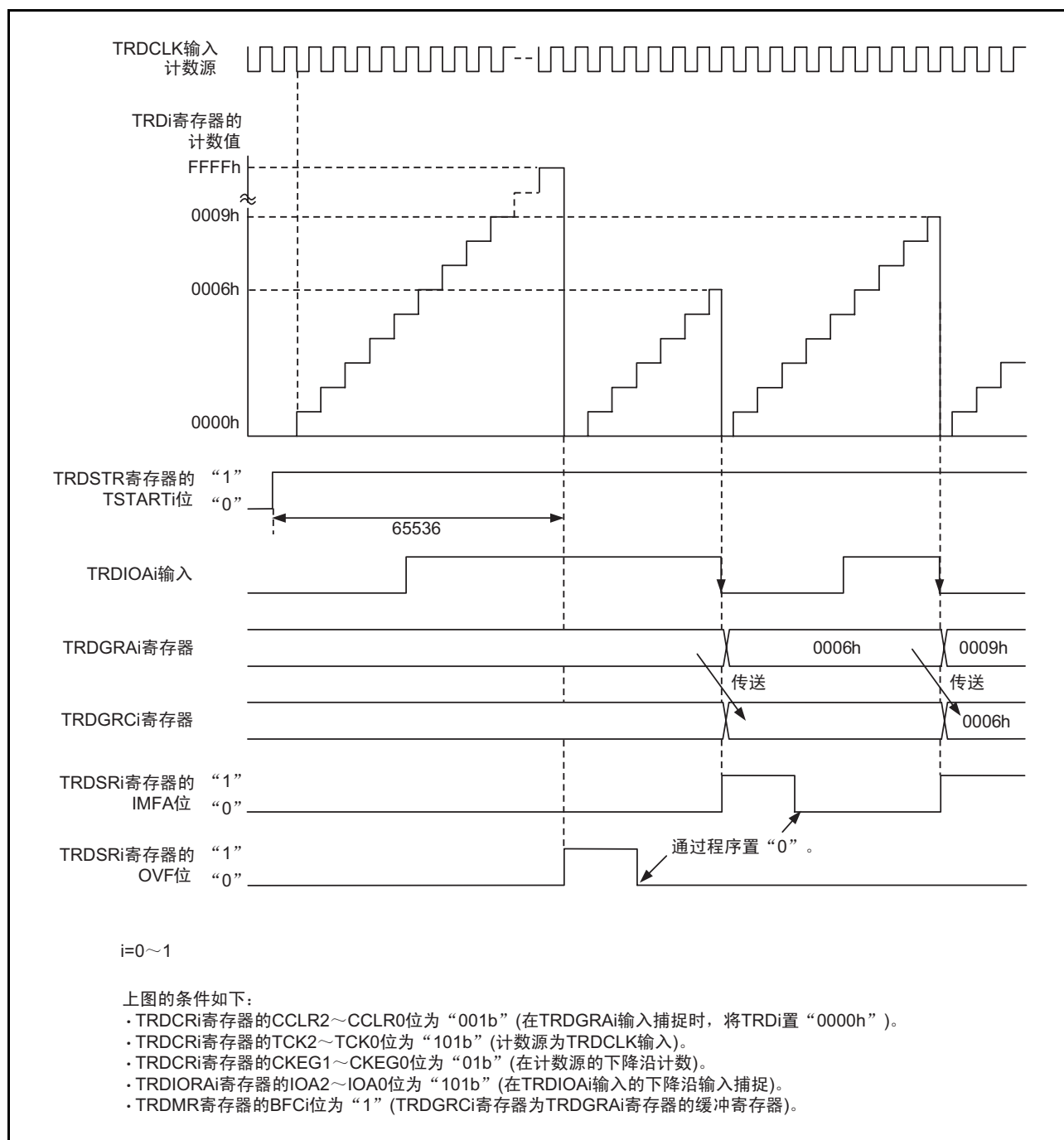
图 20.8 输入捕捉功能的运行例子
