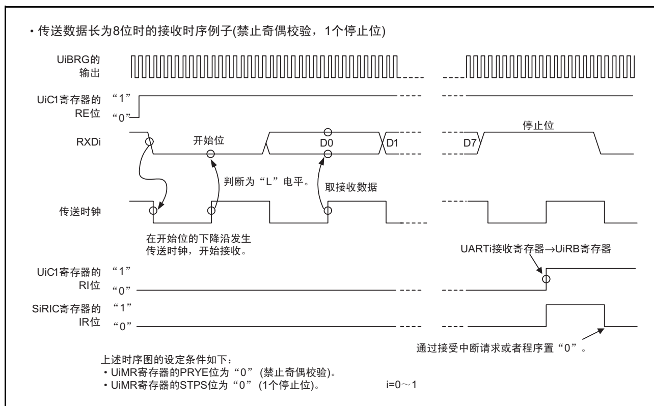
图 22.7 UART 模式的接收时序例子
