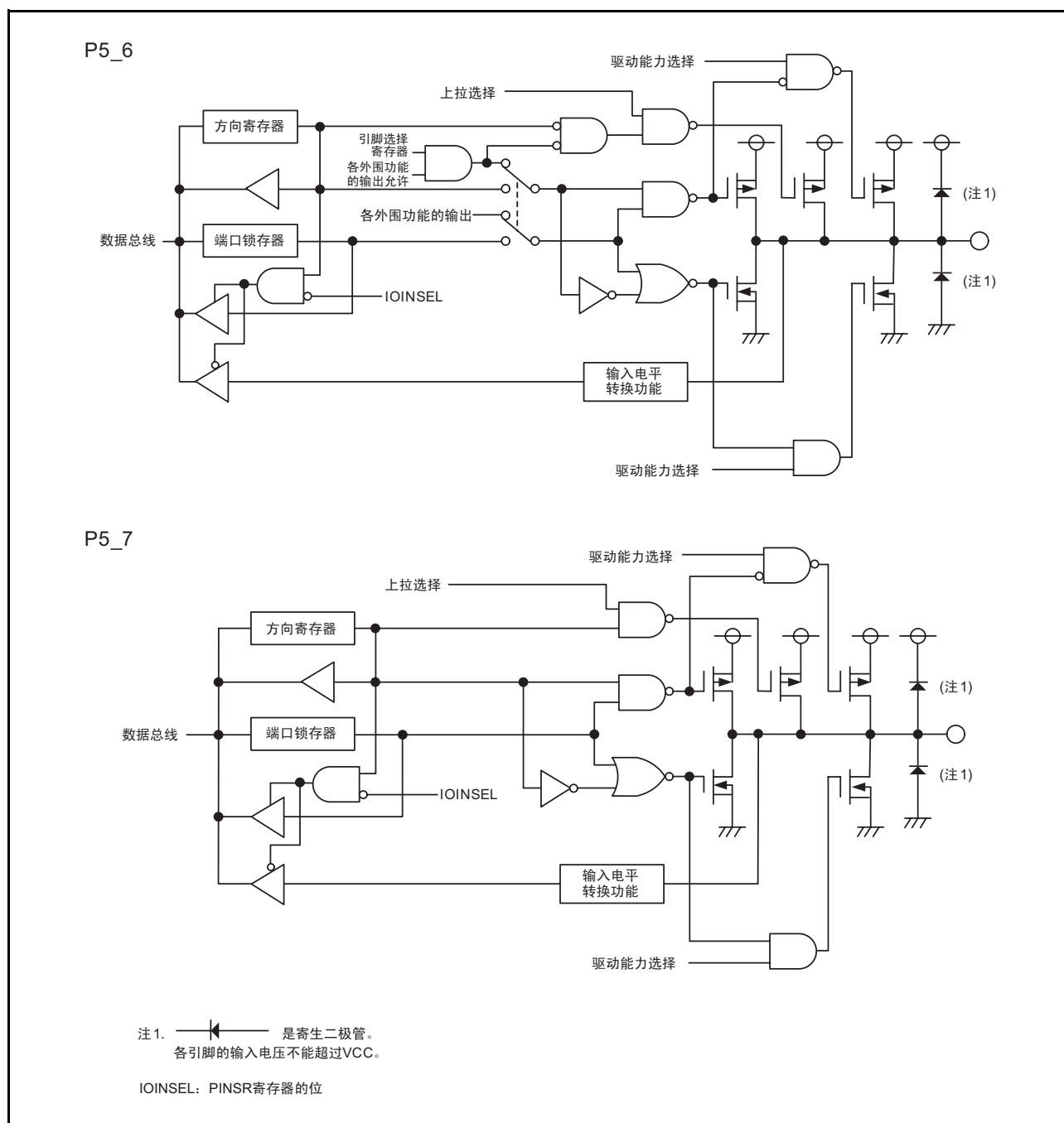
图 7.13 I/O 端口的结构 (13)
