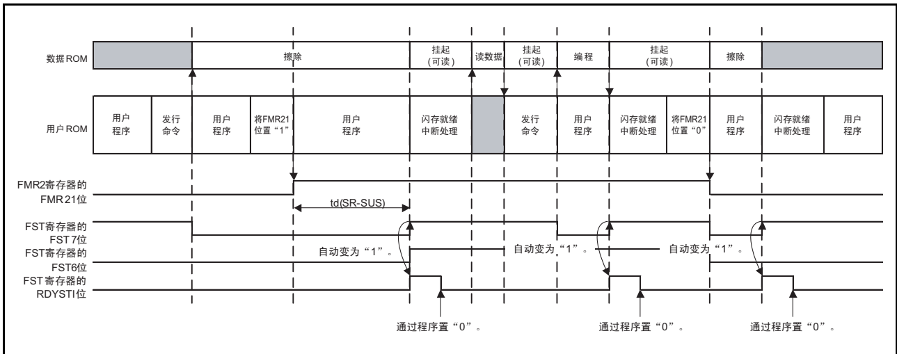
图 32.3 挂起的相关时序
