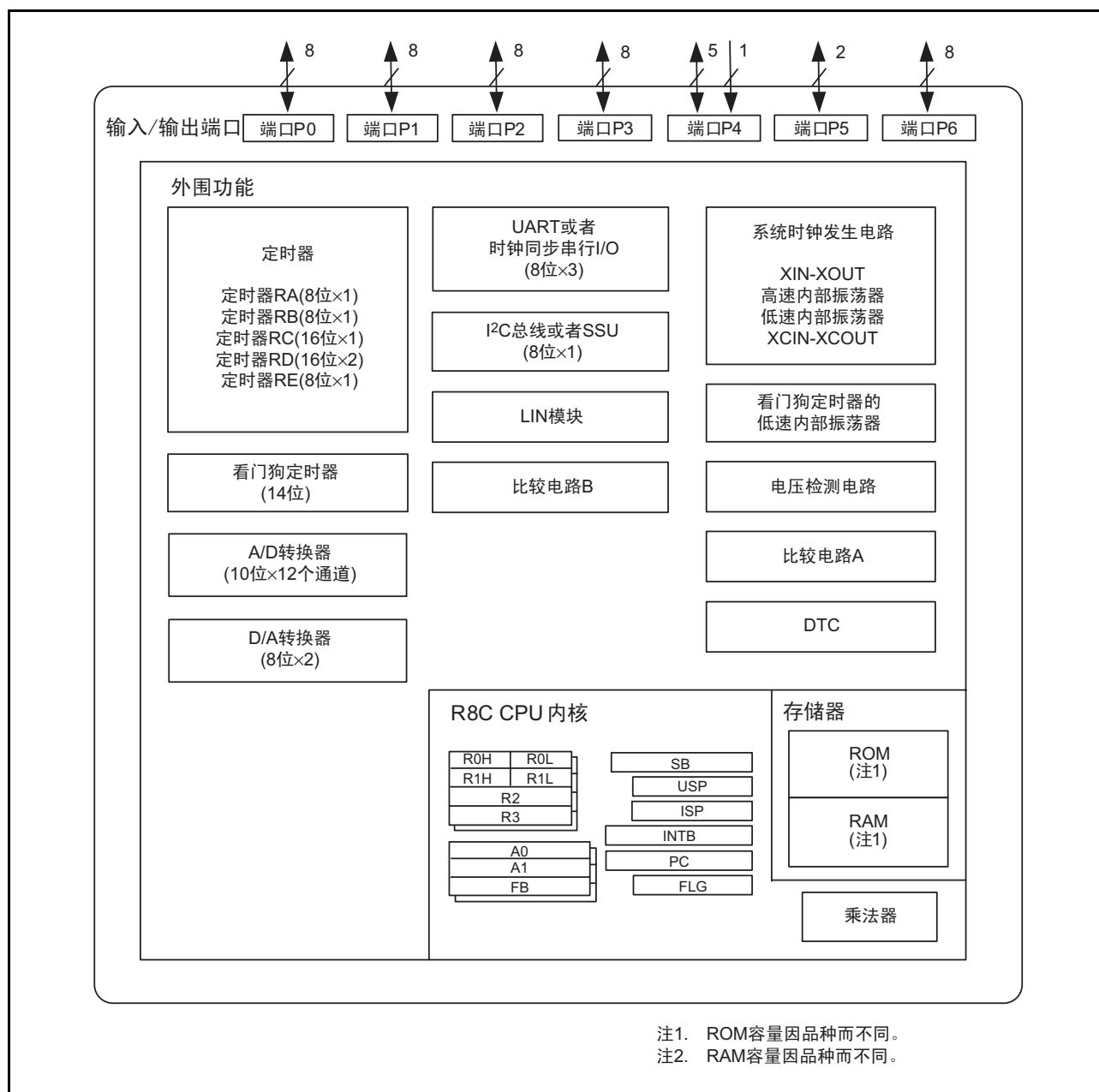
图 1.2 框图
