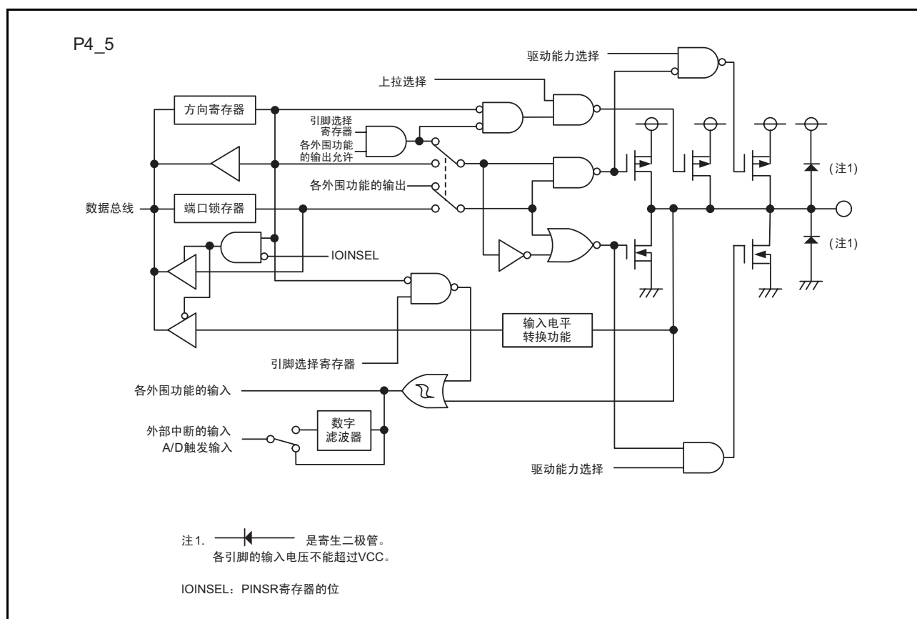
图 7.11 I/O 端口的结构 (11)
