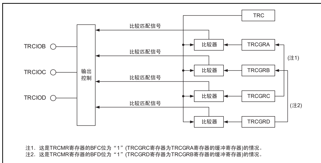
图 19.13 PWM 模式的框图
