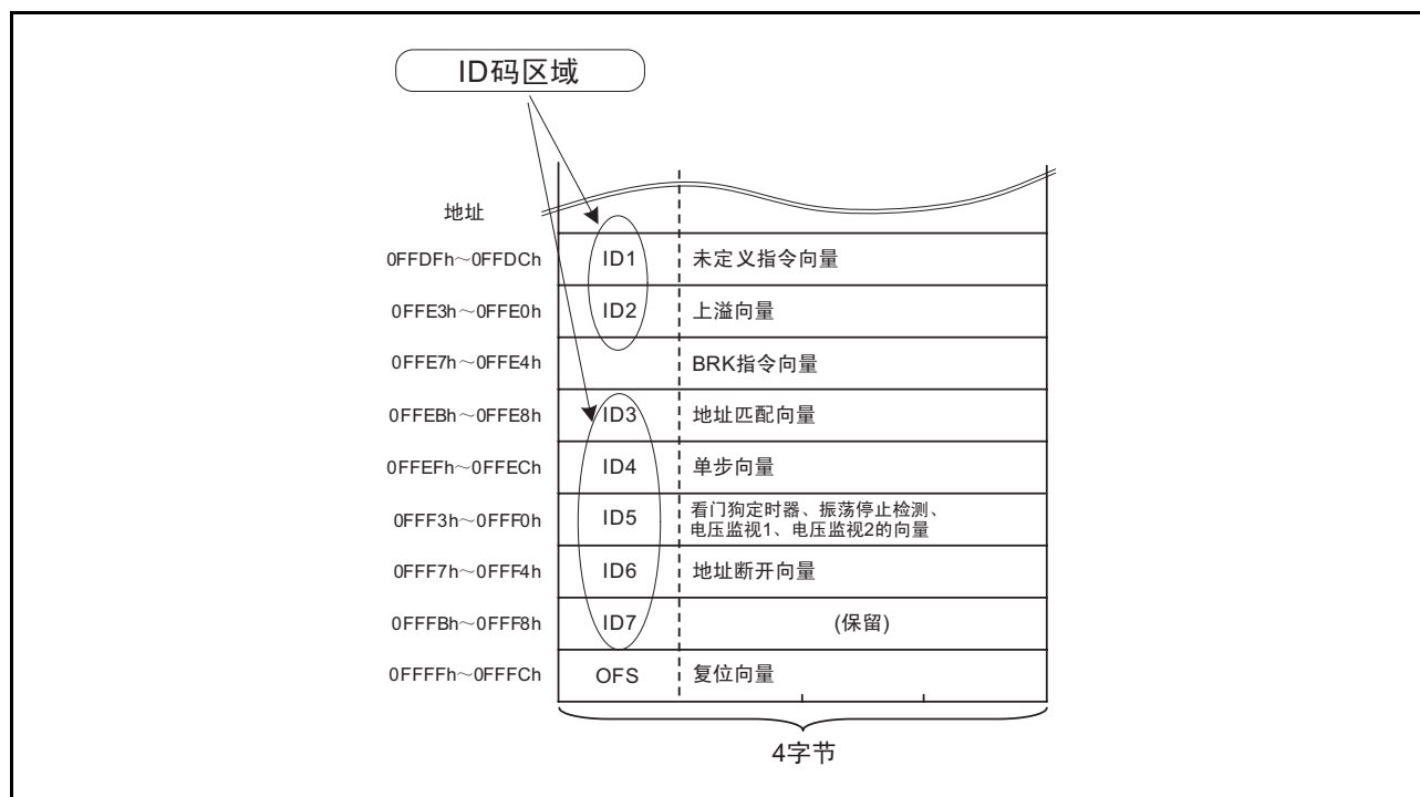
图 12.1 ID 码区域
