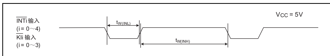
图 34.11 V_{CC}=5V 时的外部中断 \overline{INTi} 和键输入中断 \overline{Kli} 的输入时序
