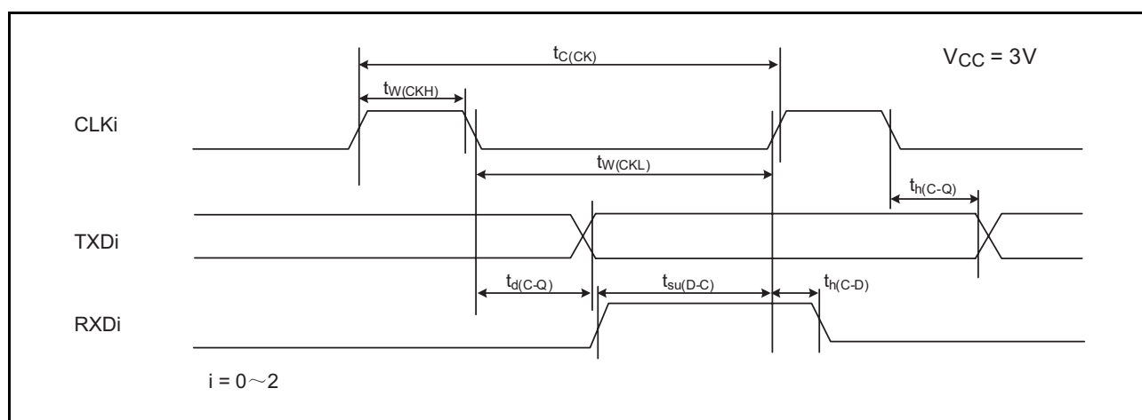
图 34.14 V_{CC}=3V 时的串行接口时序
