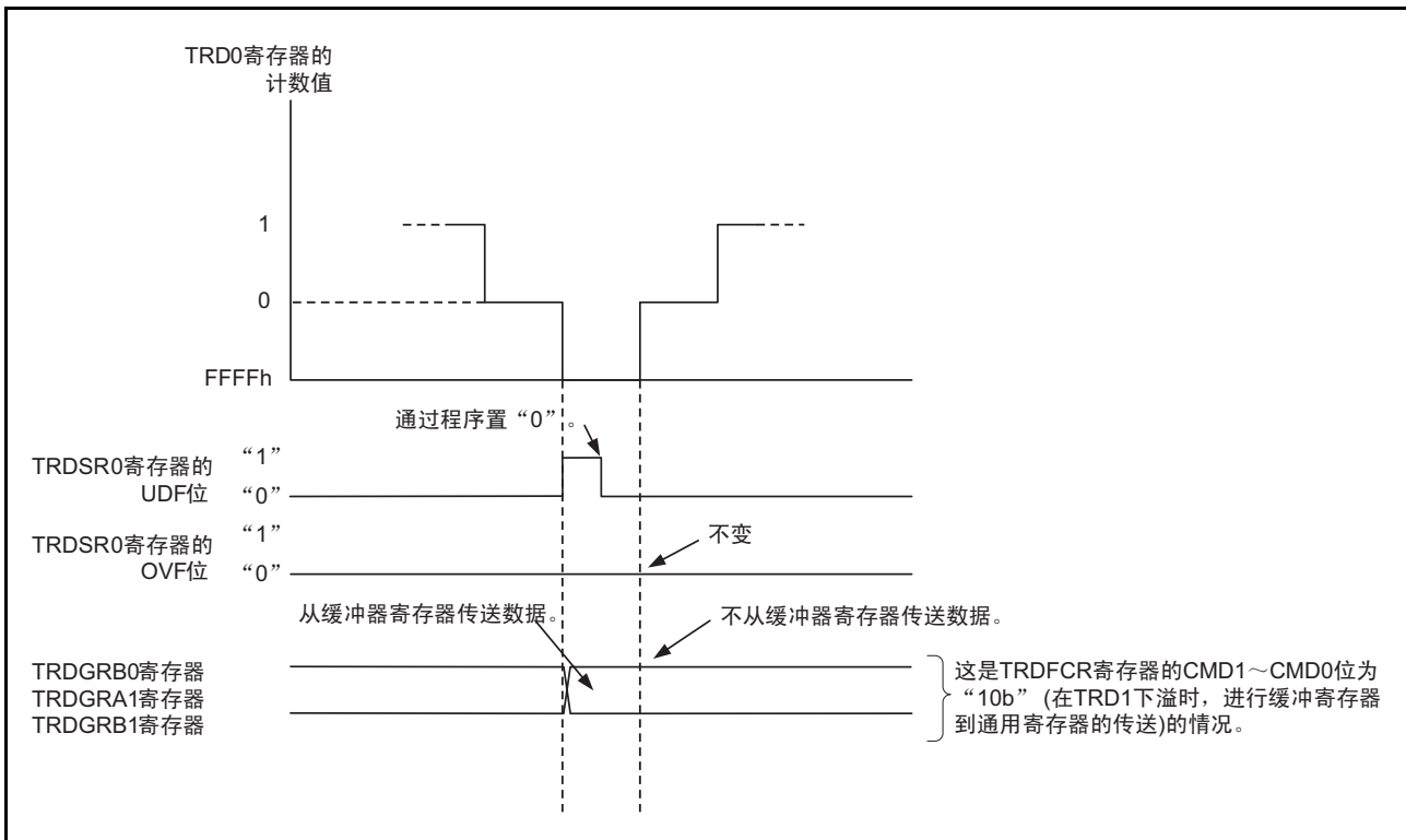
图 20.26 互补 PWM 模式中的 TRD1 发生下溢时的运行例子
