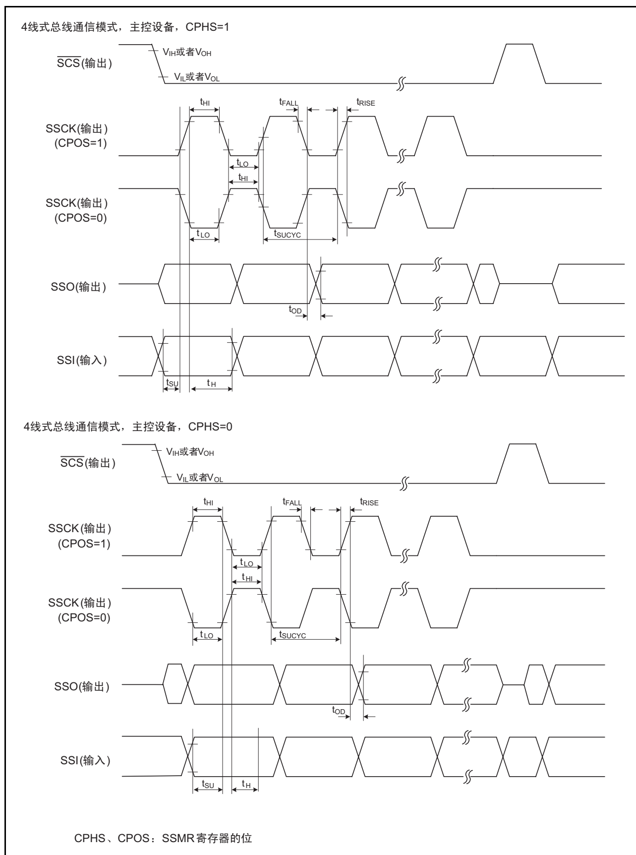
图 34.4 带片选的时钟同步串行 I/O 的输入 / 输出时序（主控制器件）
