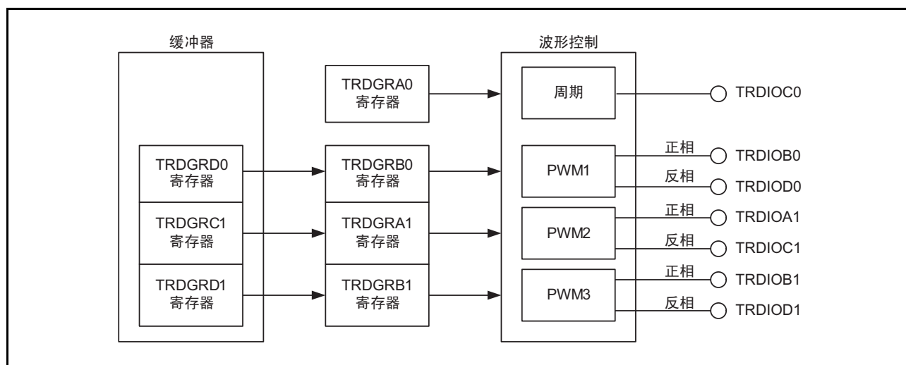
图 20.19 互补 PWM 模式的框图
