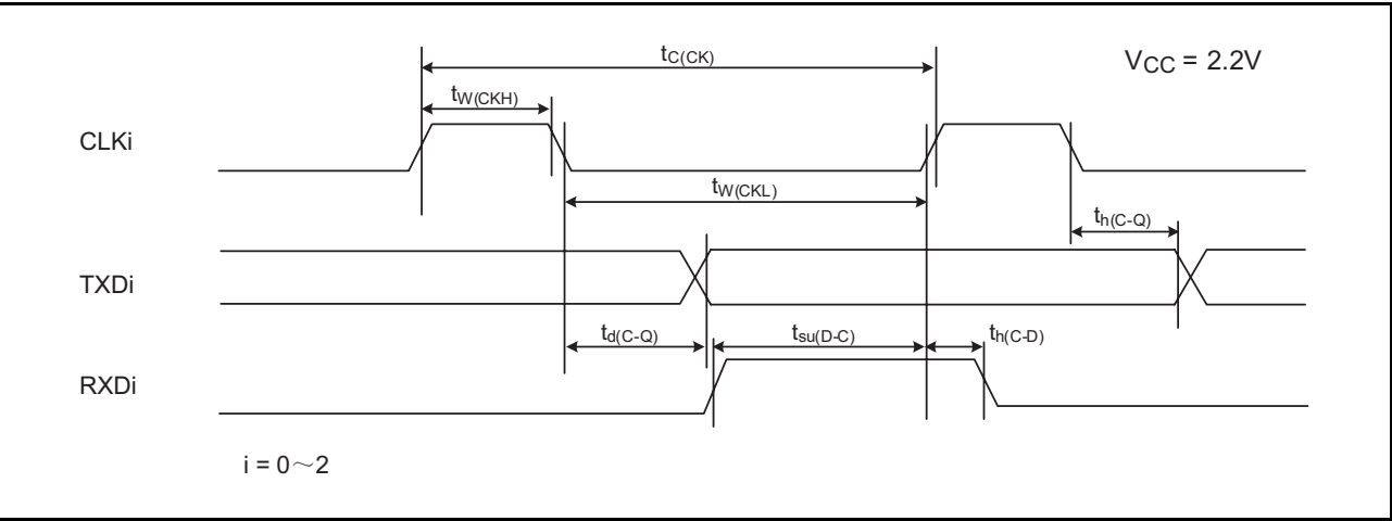
图 34.18 V_{CC}=2.2V 时的串行接口时序
