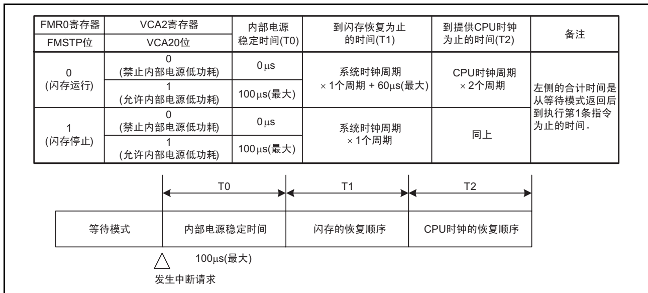
图 9.6 从 CM3 寄存器的 CM30 位被置“1”（转移到等待模式）后的等待模式到执行第 1 条指令为止的时间
