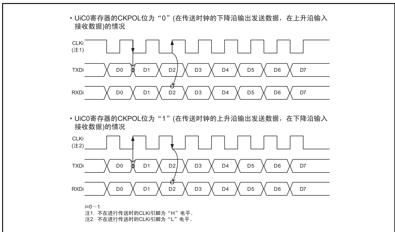
图 22.4 传送时钟的极性
