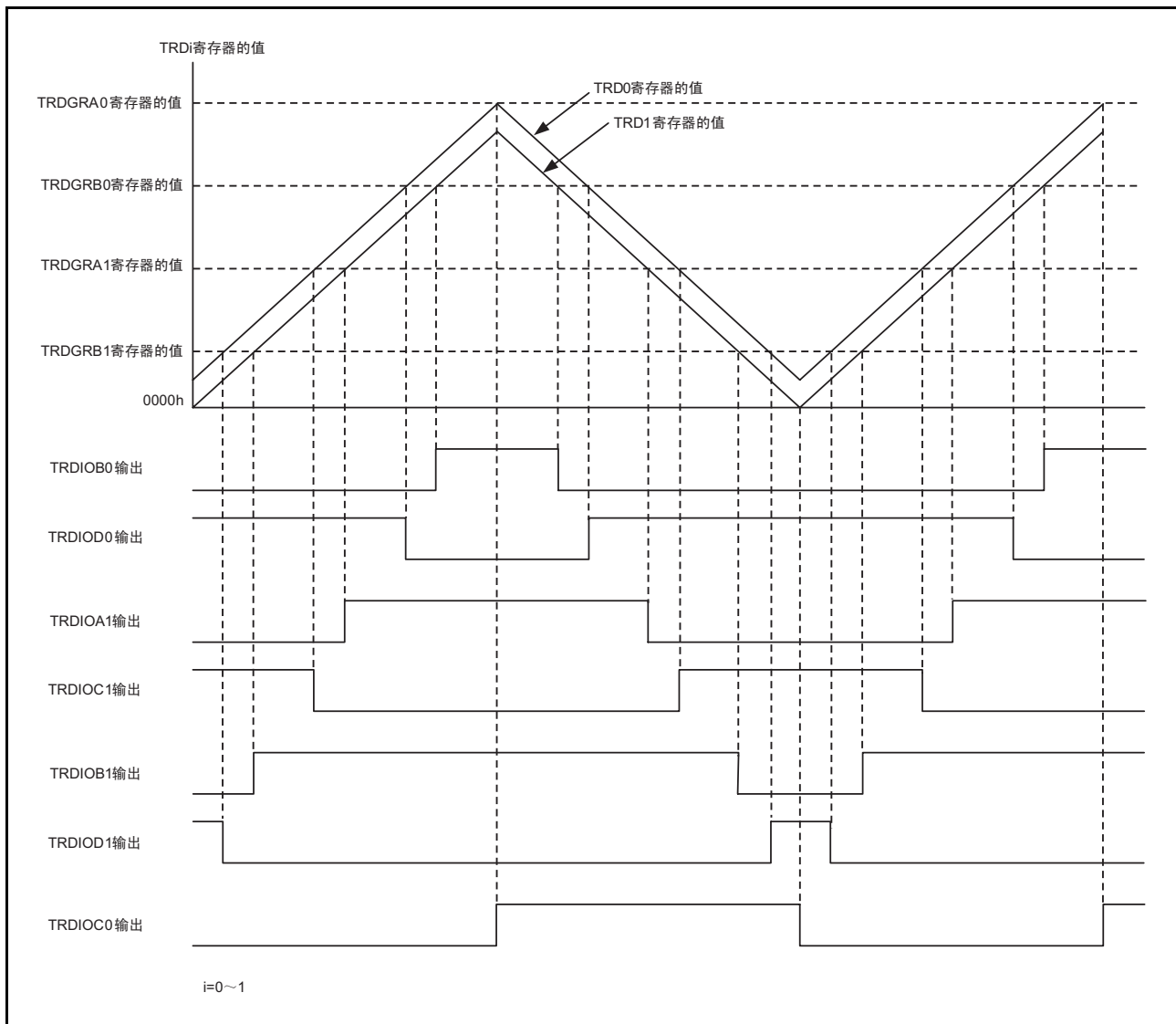
图 20.20 互补 PWM 模式的输出模型
