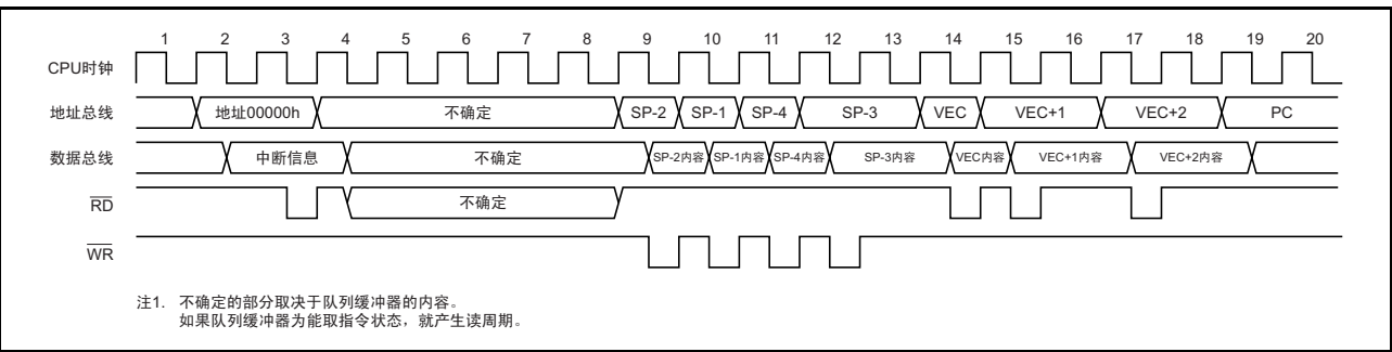
图 11.3 中断响应顺序的执行时间
