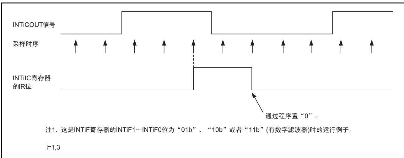
图 31.4 比较电路 Bi 数字滤波器的运行例子
