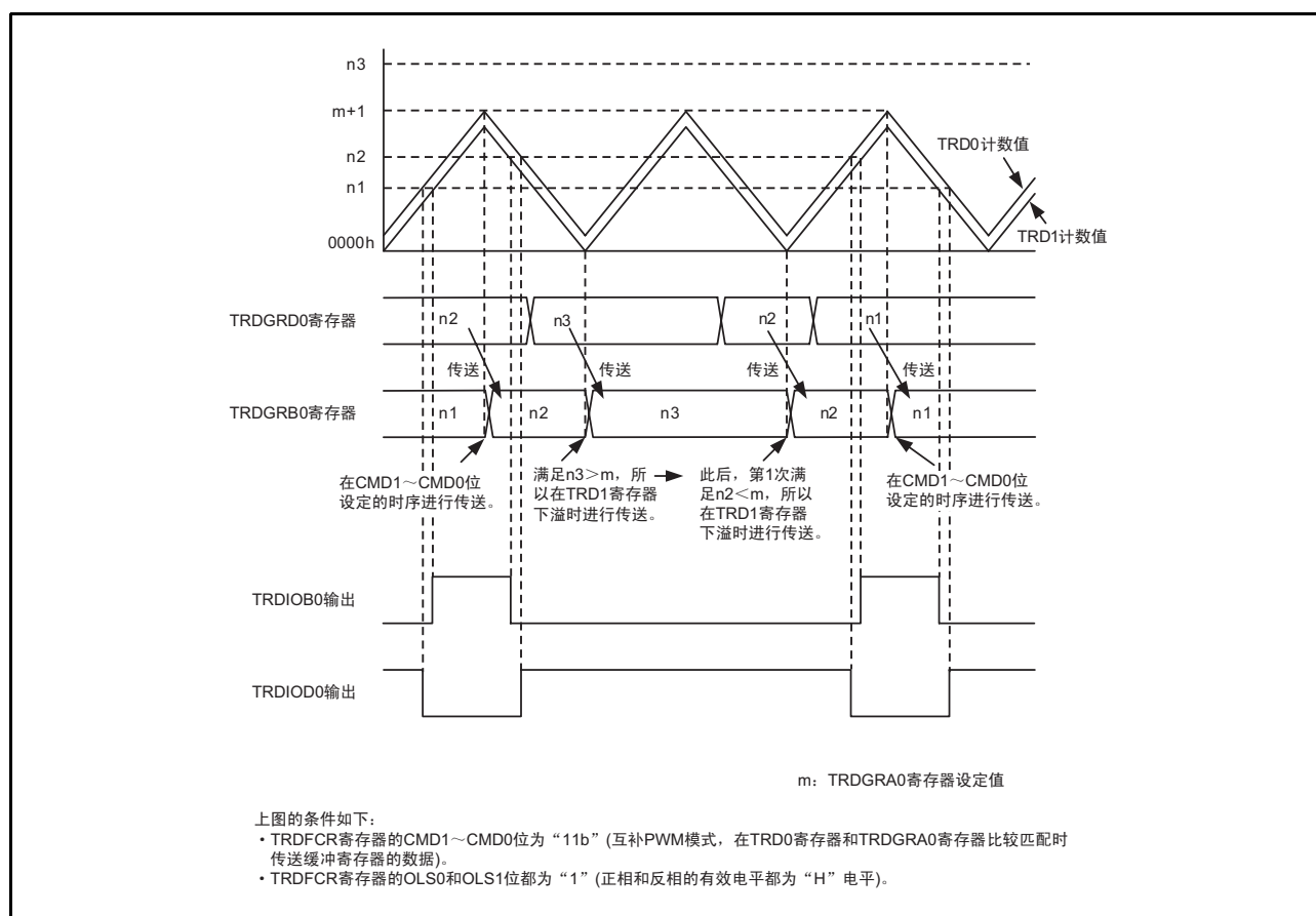
图 35.4 互补 PWM 模式中的缓冲寄存器的值 \geq TRDGRA0 寄存器的值时的运行例子
