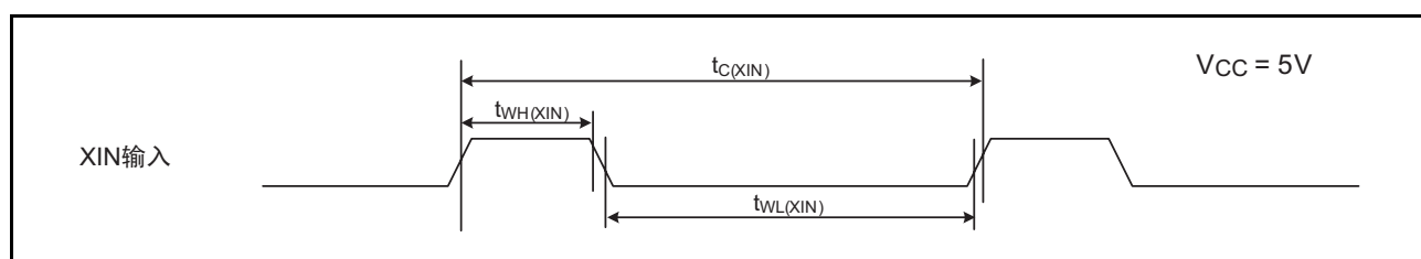
图 34.8 V_{CC}=5V 时的 XIN 和 XCIN 的输入时序
