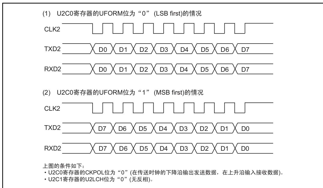
图 23.5 传送格式
