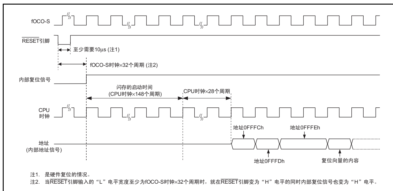
图 5.3 复位顺序
