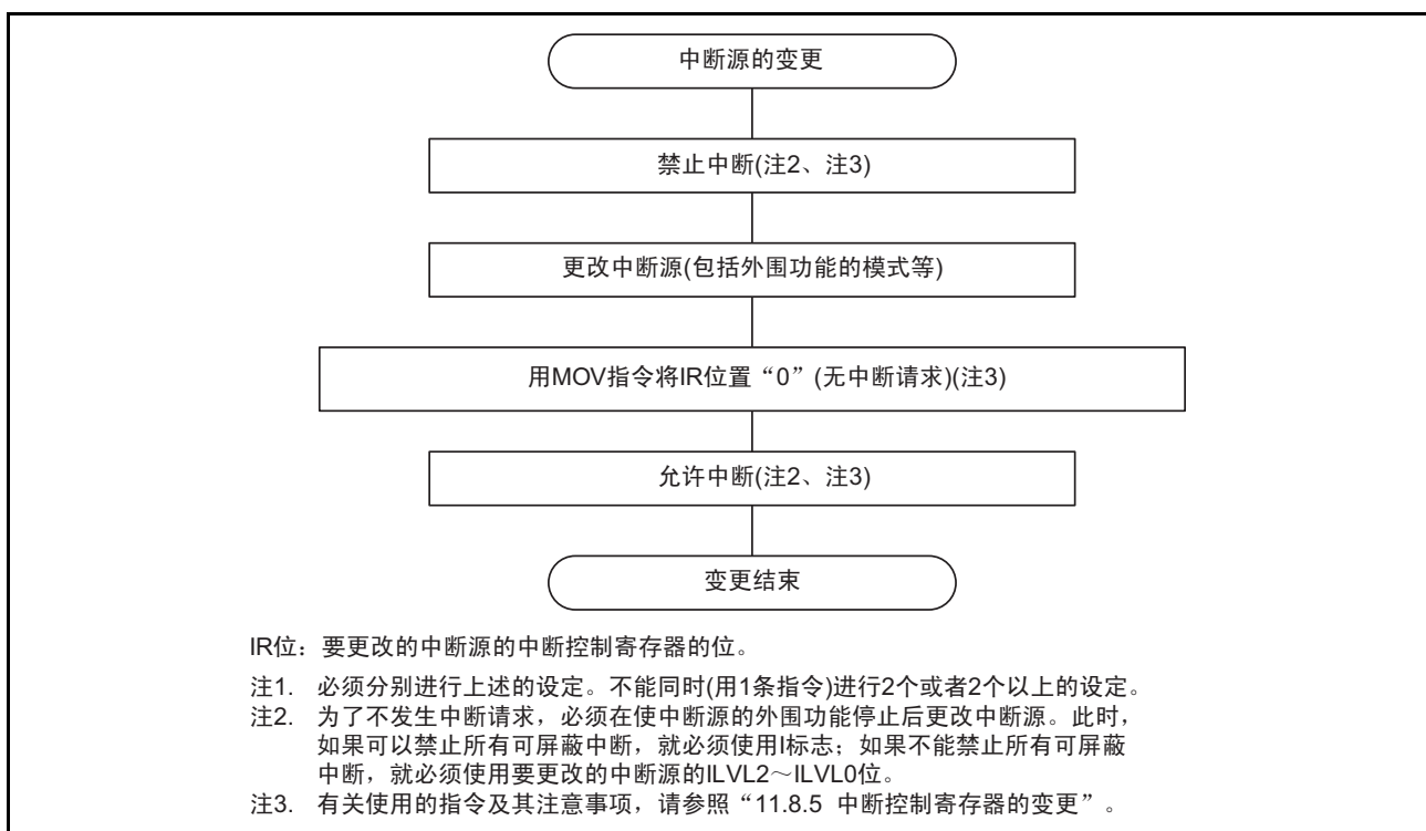
图 11.13 中断源的变更步骤例子
