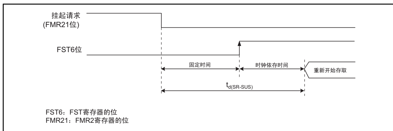
图 34.2 挂起的转移时间
