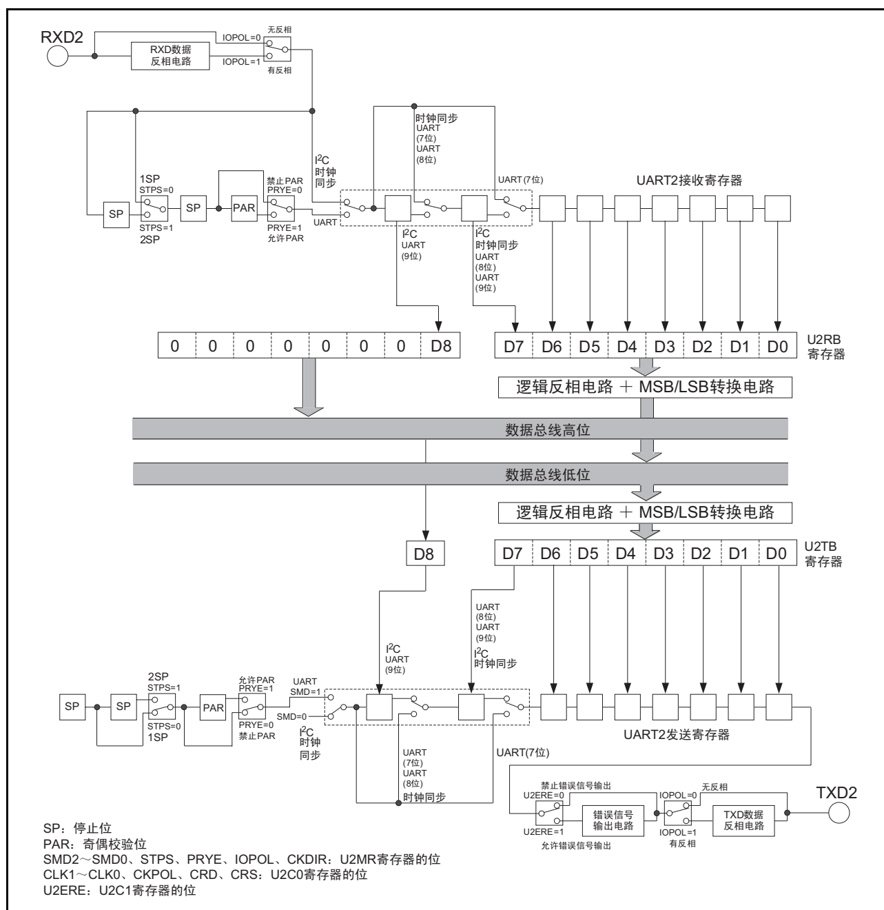
图 23.2 UART2 发送 / 接收部的框图
