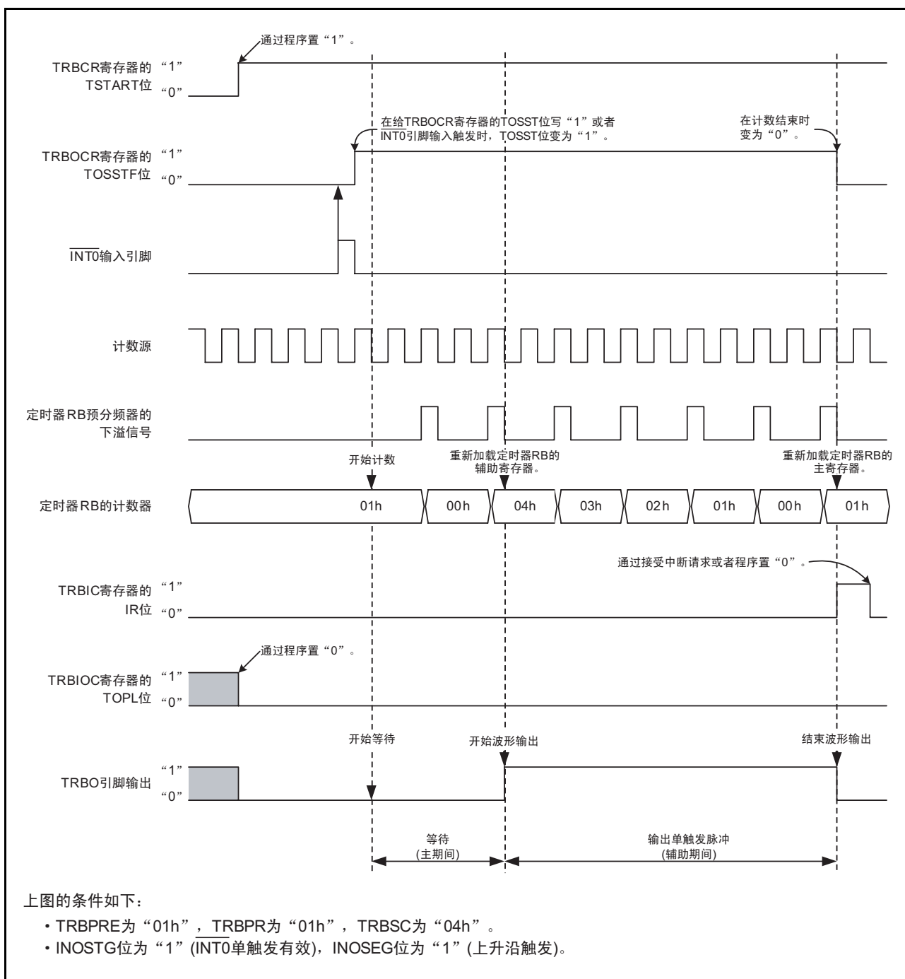
图 18.5 可编程等待单触发生模式的运行例子
