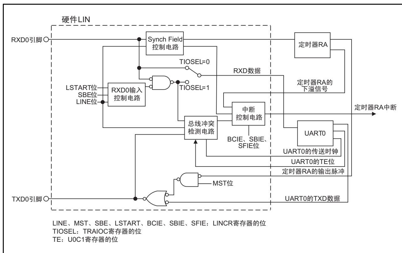
图 27.1 硬件 LIN 的框图
