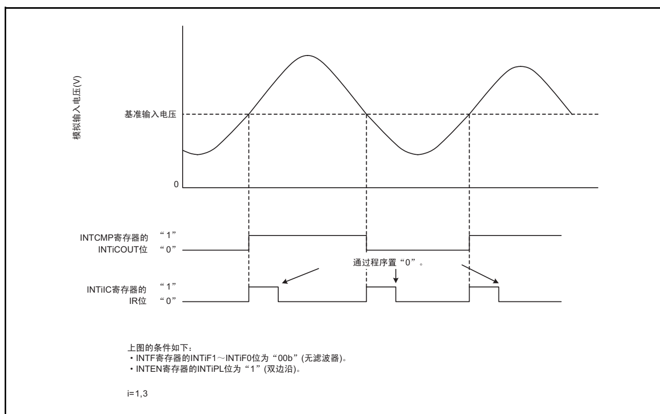
图 31.2 比较电路 Bi（i=1,3）的运行例子
