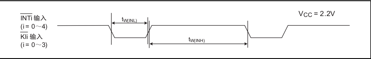
图 34.19 V_{CC}=2.2V 时的外部中断 \overline{INTi} 和键输入中断 \overline{Kli} 的输入时序
