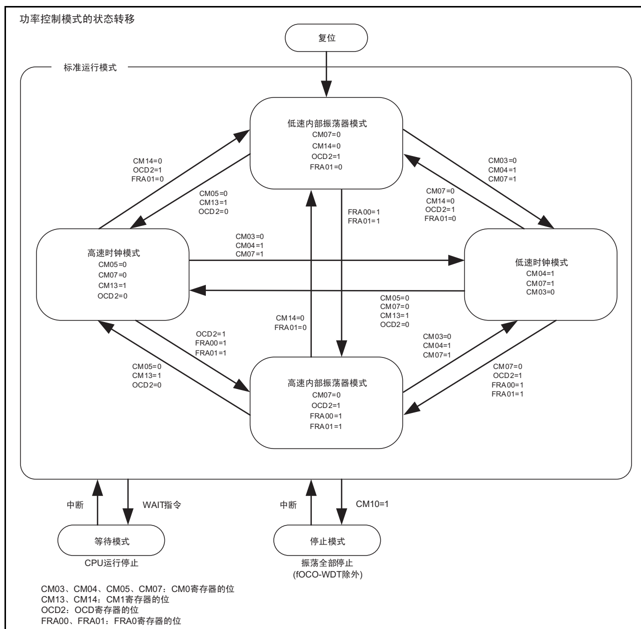
图 9.9 功率控制模式的状态转移
