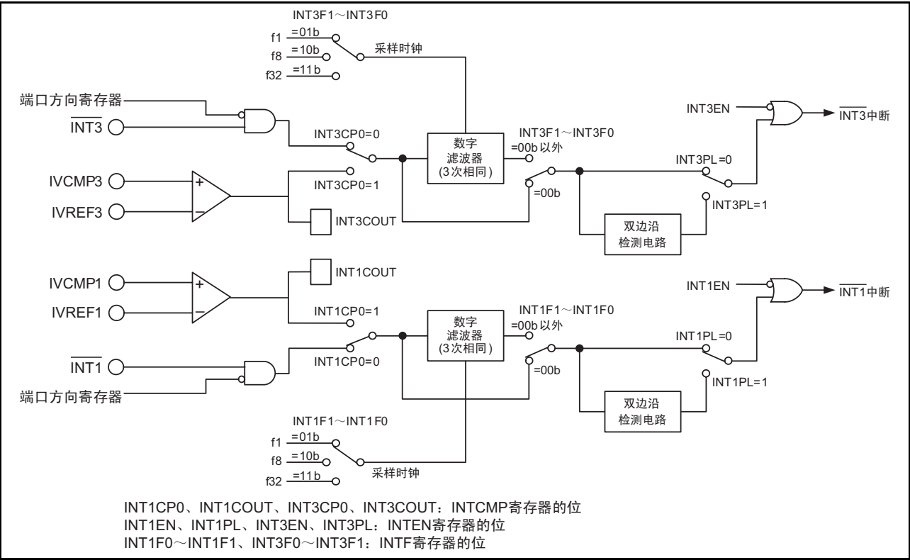
图 31.1 比较电路 B 的框图
