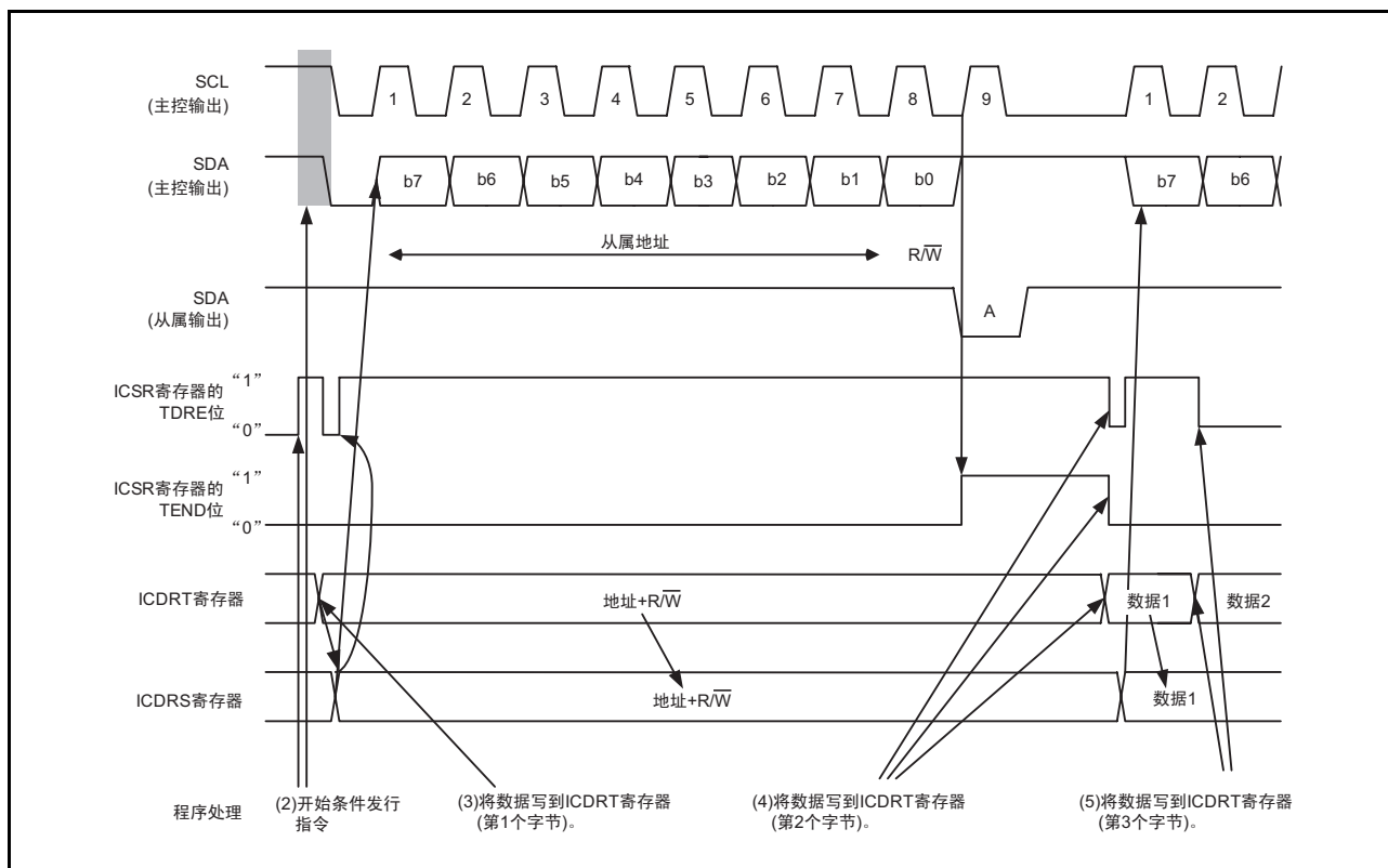
图 26.5 主控发送模式的运行时序（I 2 C 总线接口模式）（1）
