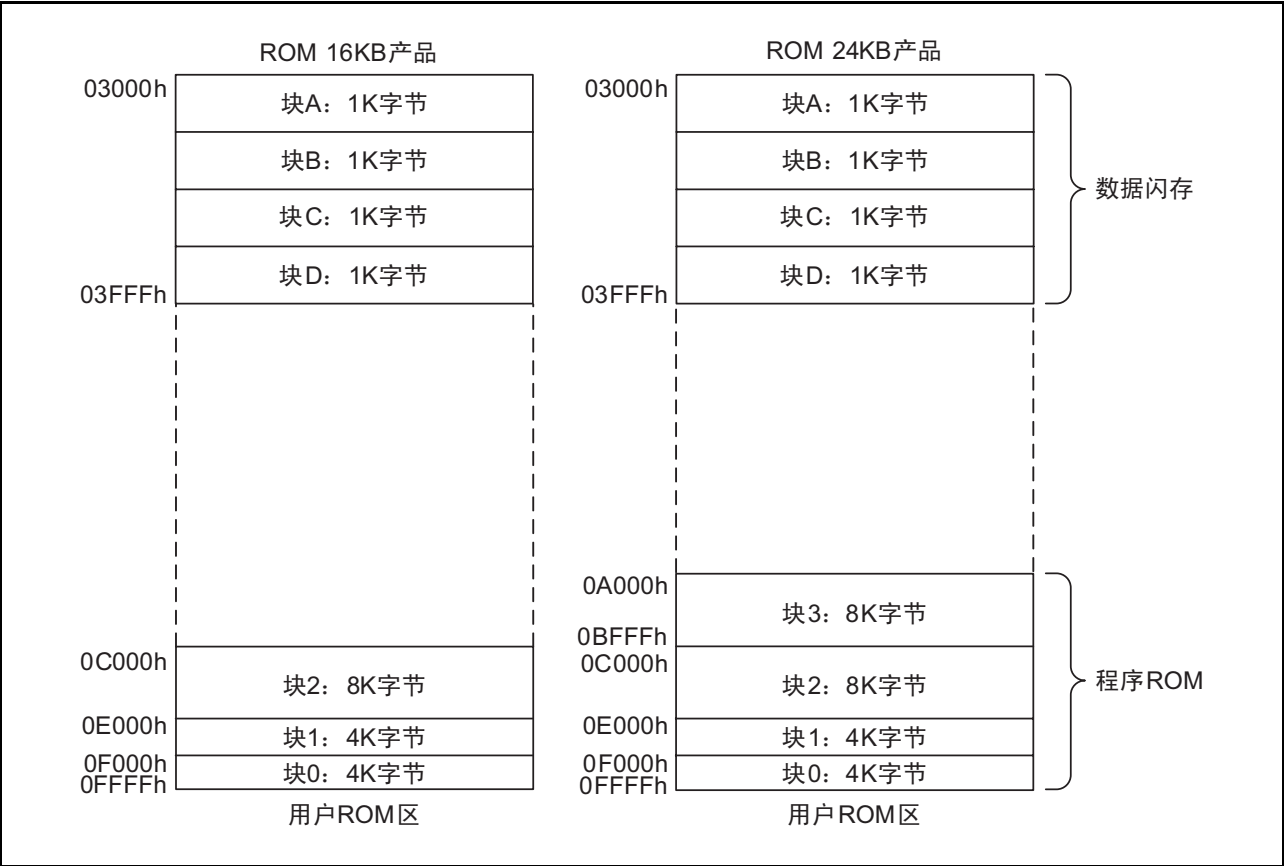
图 32.1 R8C/35A 群的闪存框图（1）
