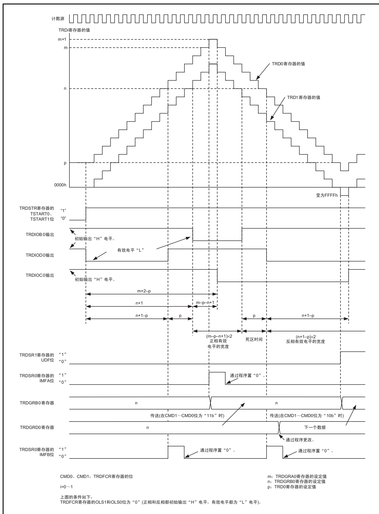
图 20.21 互补 PWM 模式的运行例子
