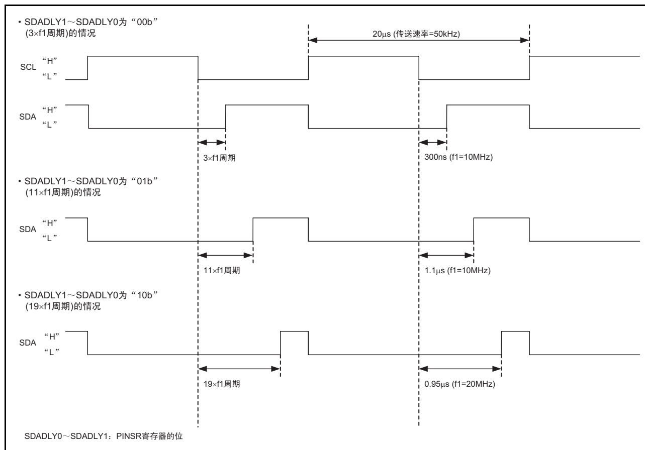
图 26.3 SDA 引脚的数字延迟的运行例子
