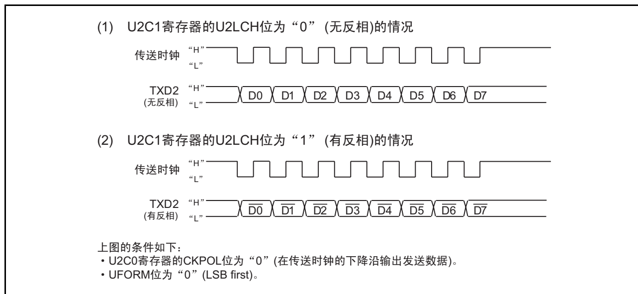
图 23.6 串行数据的逻辑
