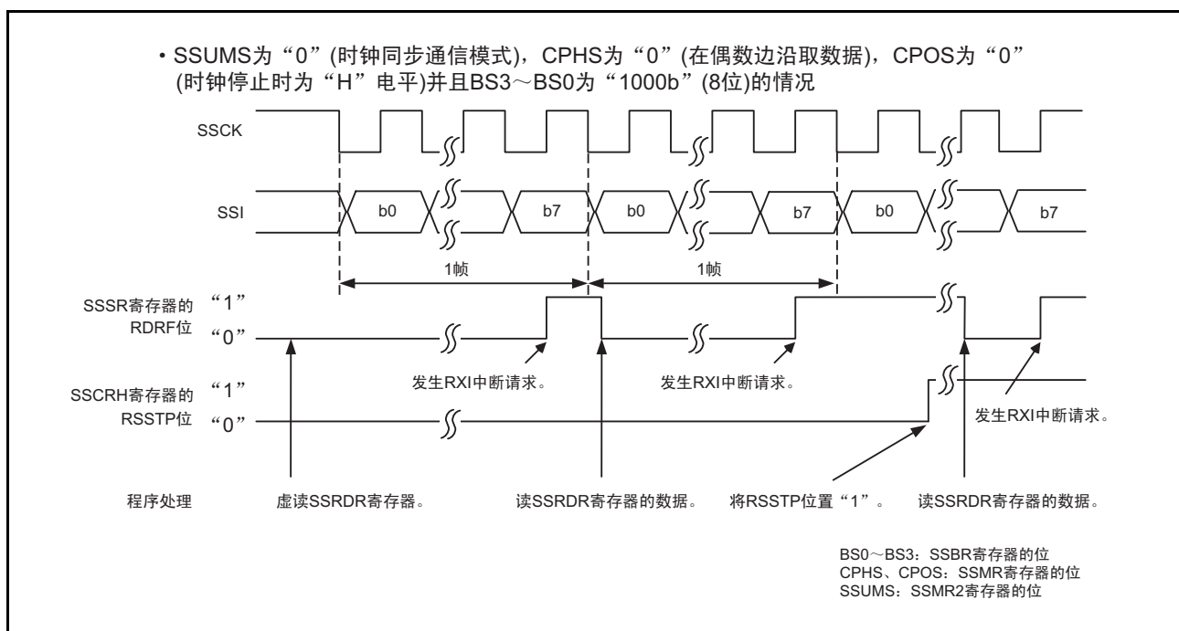
图 25.7 接收数据时的运行例子（时钟同步通信模式、SSU 数据传送长度为 8 位）
