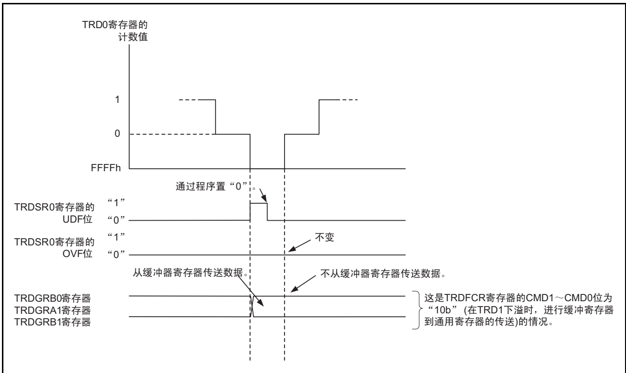
图 35.3 互补 PWM 模式中的 TRD1 发生下溢时的运行例子
