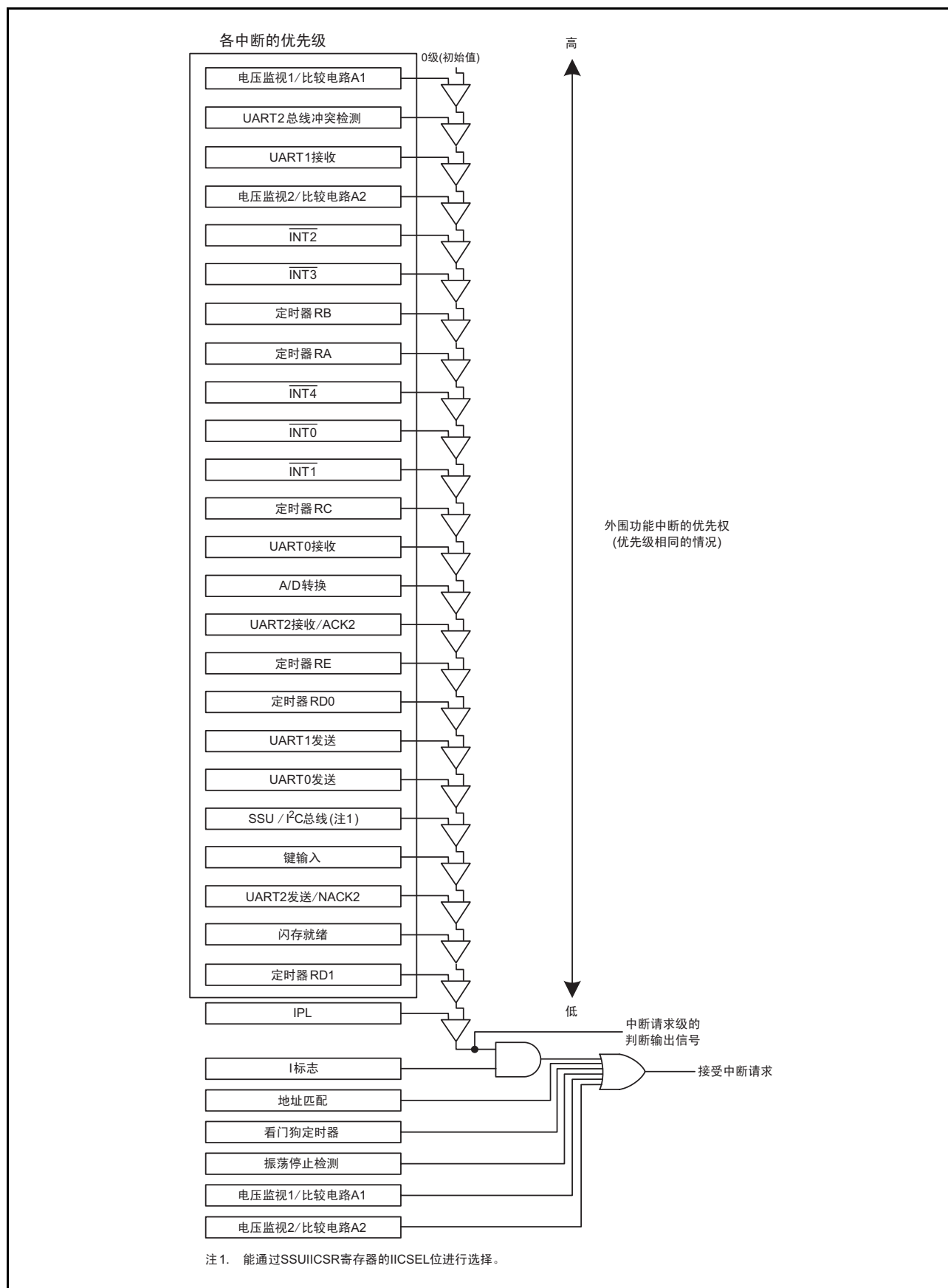
图 11.8 中断优先级的判断电路
