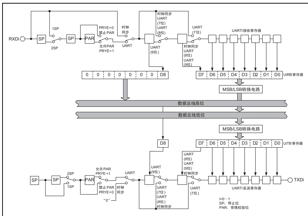
图 22.2 发送 / 接收部的框图
