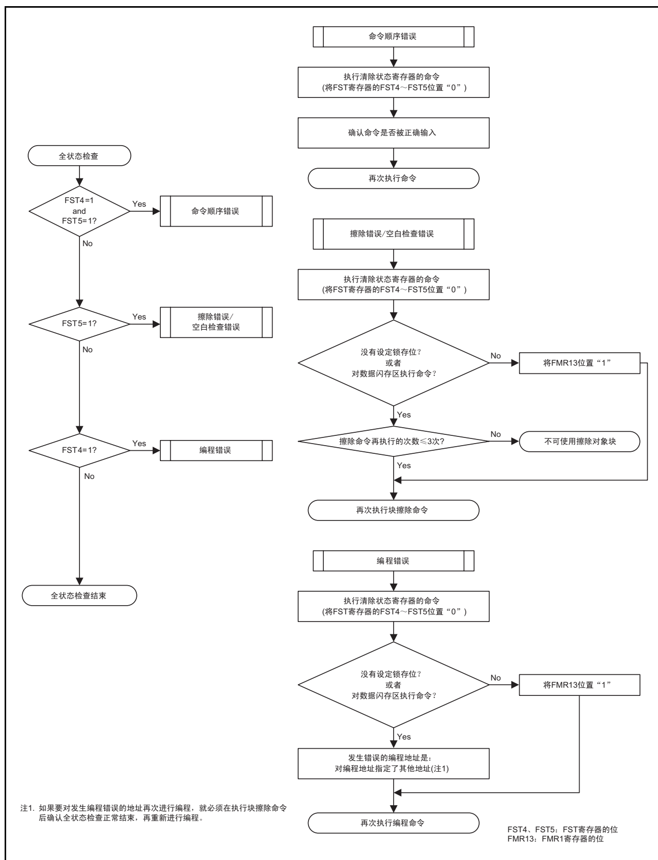
图 32.16 全状态检查的流程图和发生各错误时的处理方法
