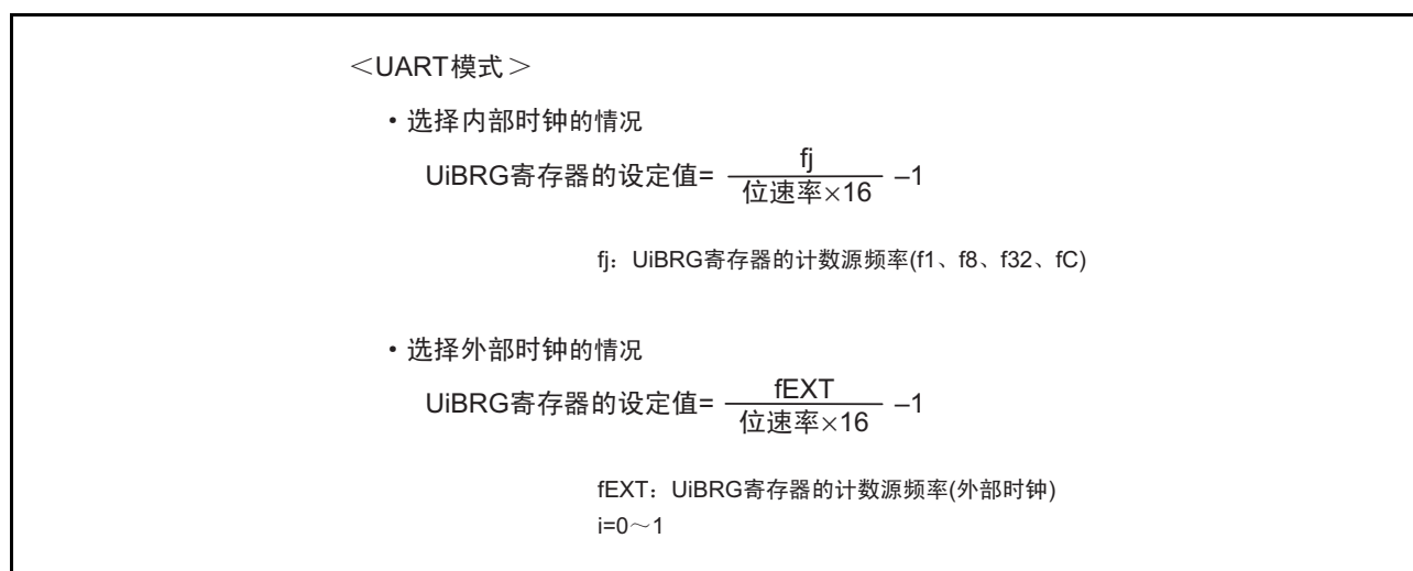
图 22.8 UiBRG 寄存器 (i=0 ~ 1) 的设定值的计算式
