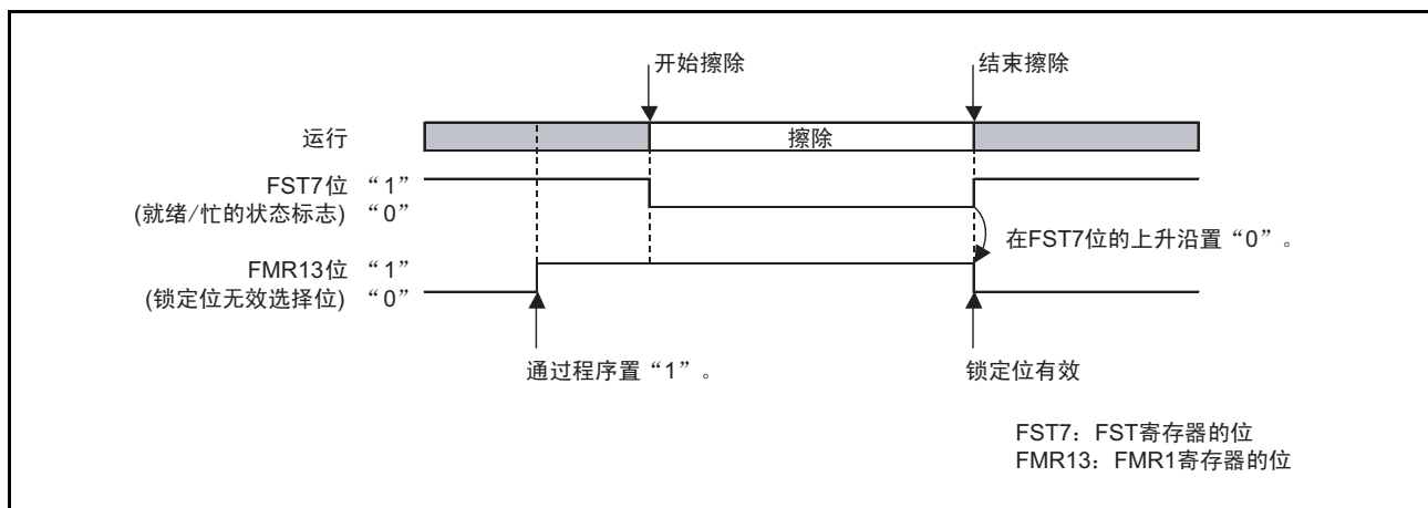
图 32.7 FMR13 位操作的相关时序
