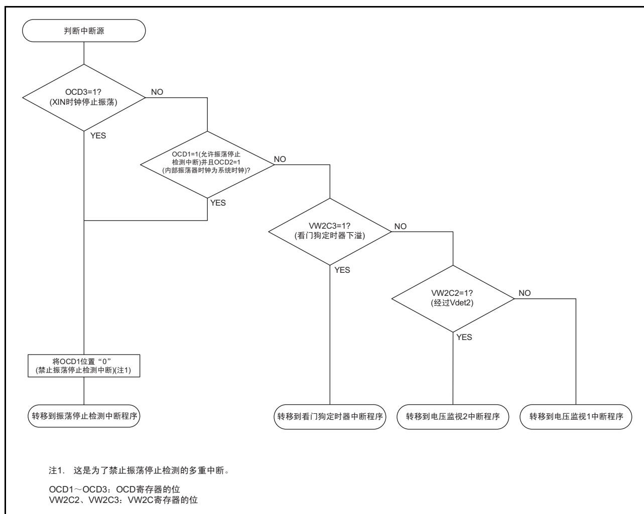
图 9.11 振荡停止检测中断、看门狗定时器中断、电压监视 1 中断和电压监视 2 中断的中断源判断方法的例子
