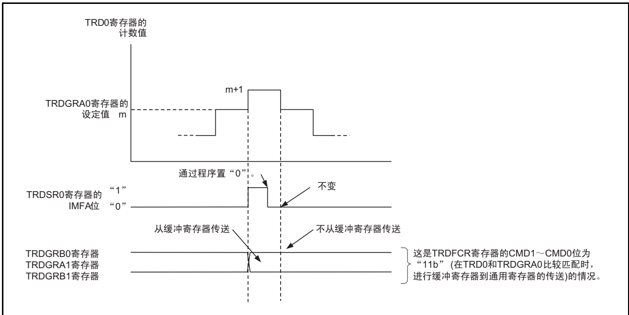
图 35.2 互补 PWM 模式中的 TRD0 和 TRDGRA0 寄存器比较匹配时的运行例子
