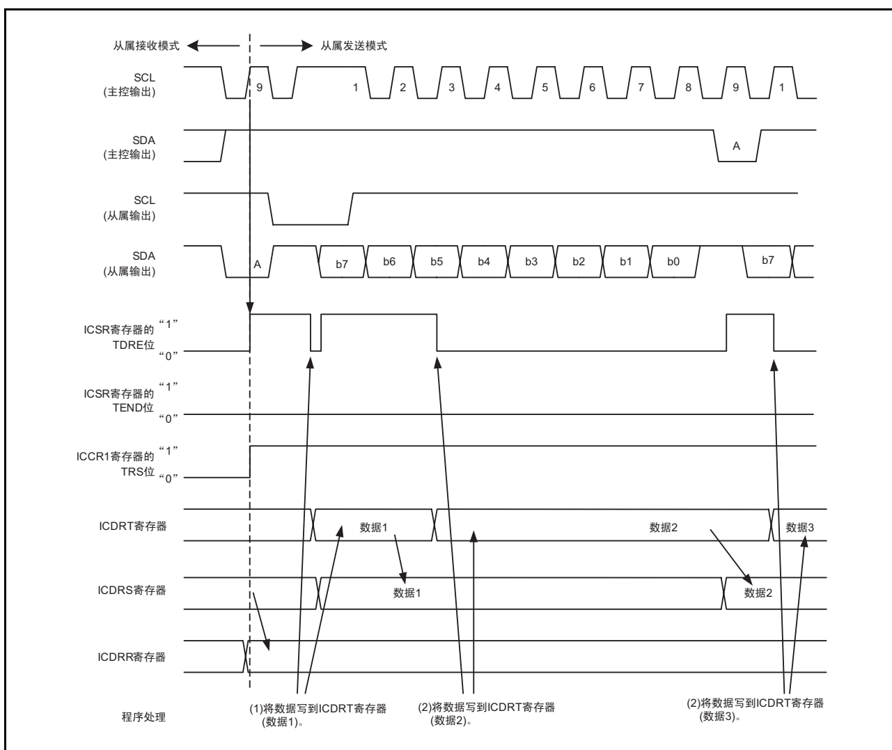
图 26.9 从属发送模式的运行时序 (I 2 C 总线接口模式) (1)
