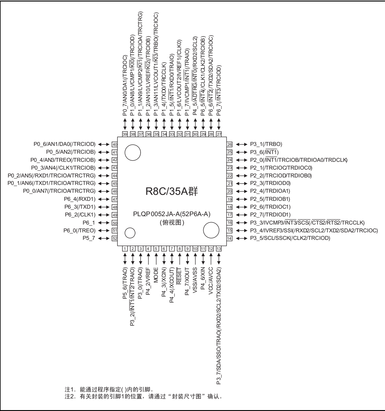
图 1.3 引脚排列图（俯视图）
