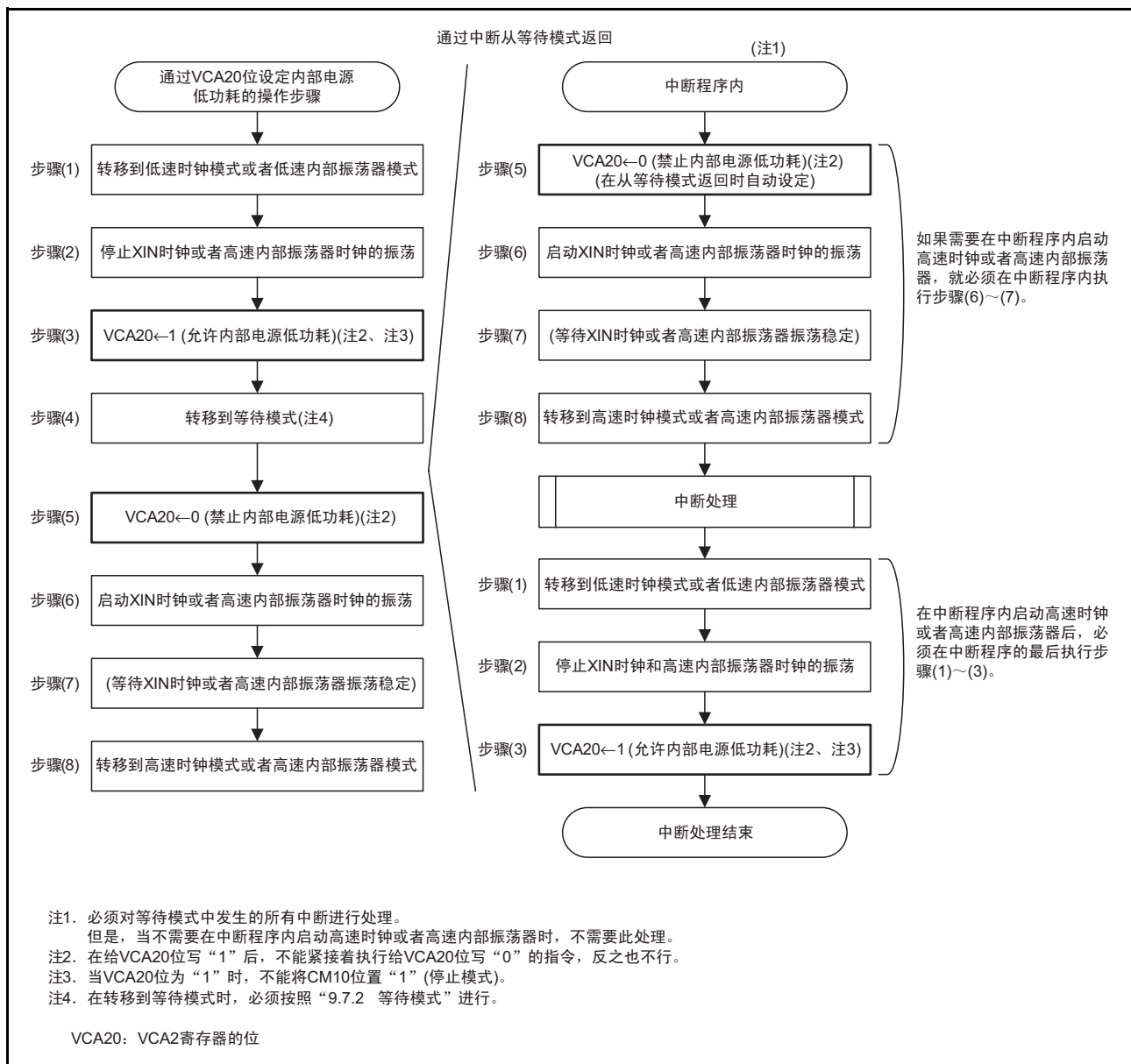
图 33.1 通过 VCA20 位设定内部电源低功耗的操作步骤
