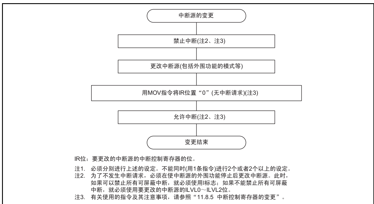
图 35.1 中断源的变更步骤例子
