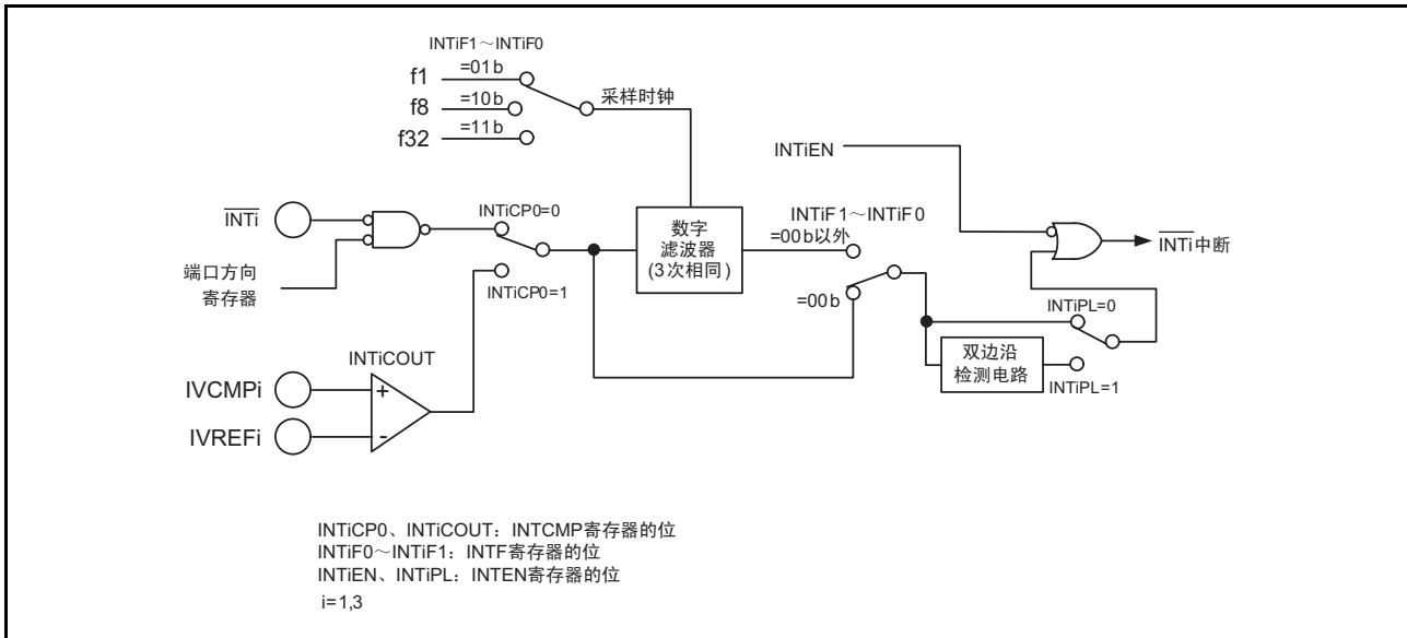
图 31.3 比较电路 Bi 数字滤波器的结构
