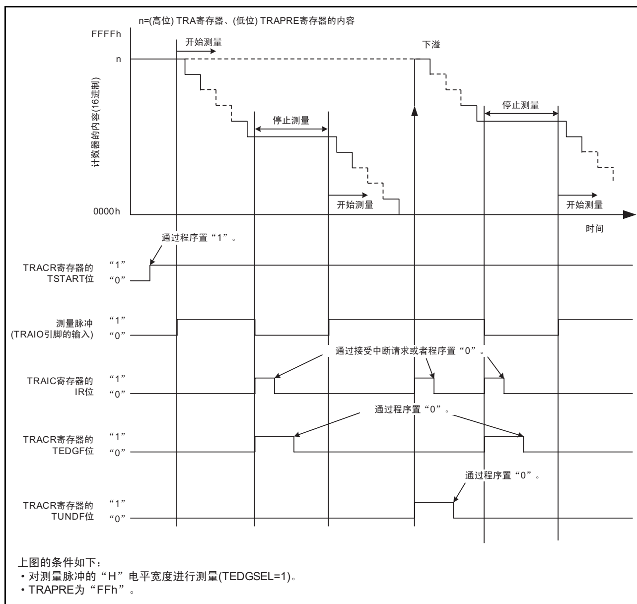
图 17.3 脉宽测量模式的运行例子
