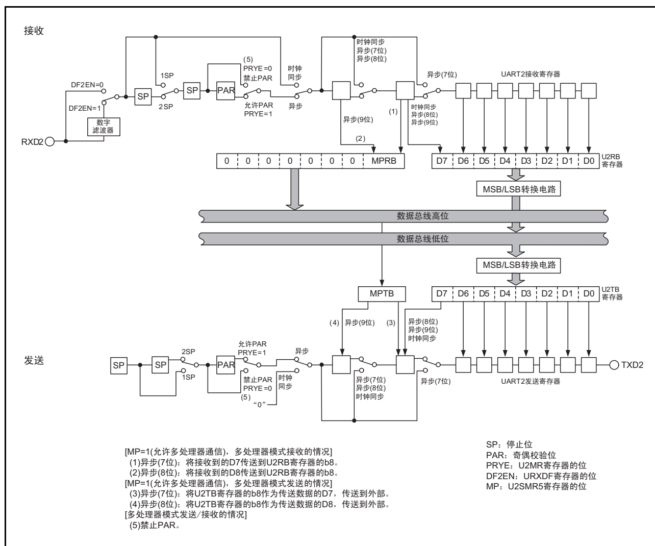
图 23.18 多处理器通信功能的框图
