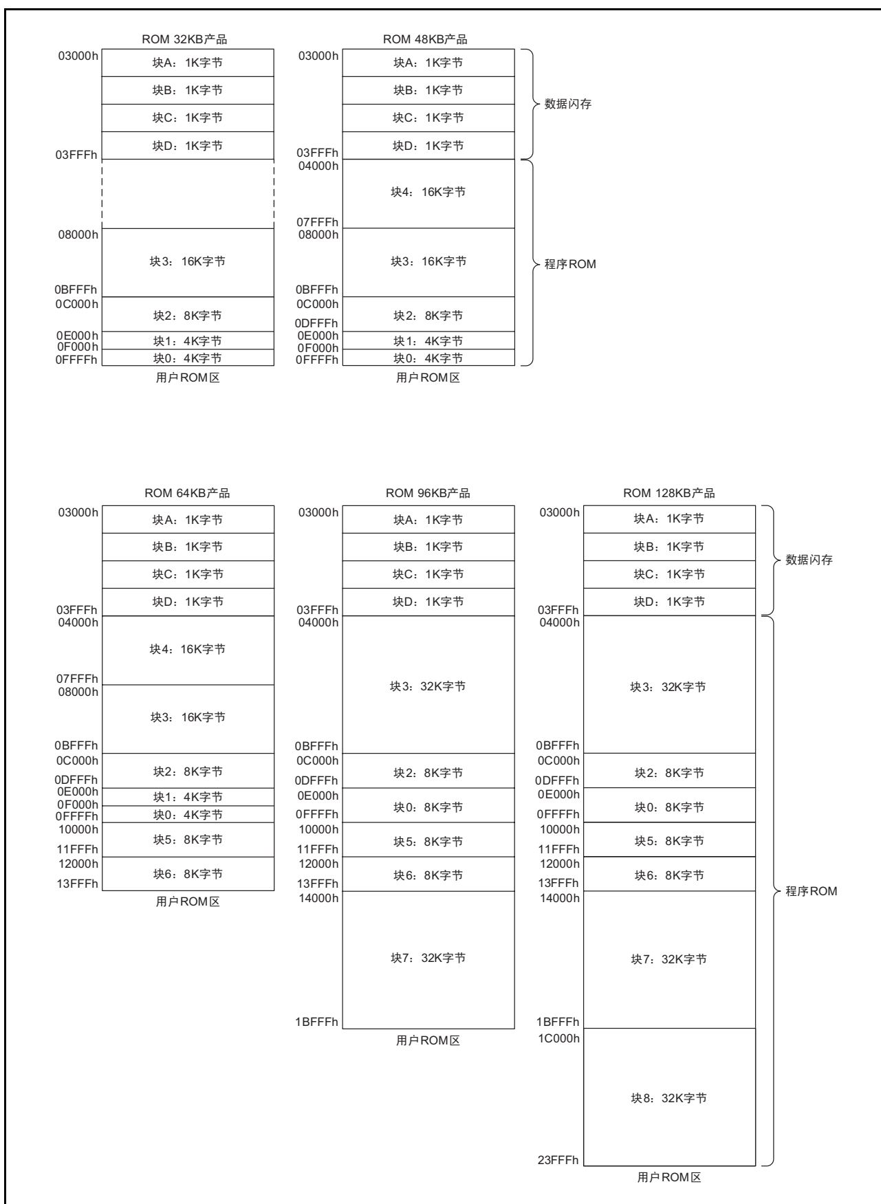
图 32.2 R8C/35A 群的闪存框图 (2)
