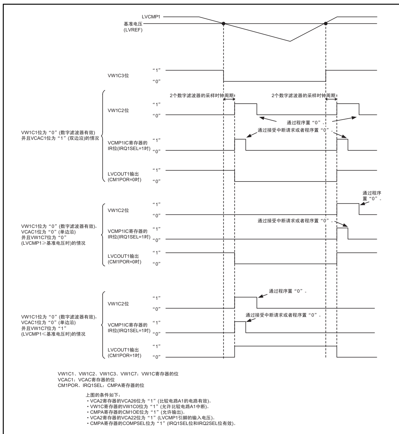
图 30.2 比较电路 A1 的运行例子 (数字滤波器有效)
