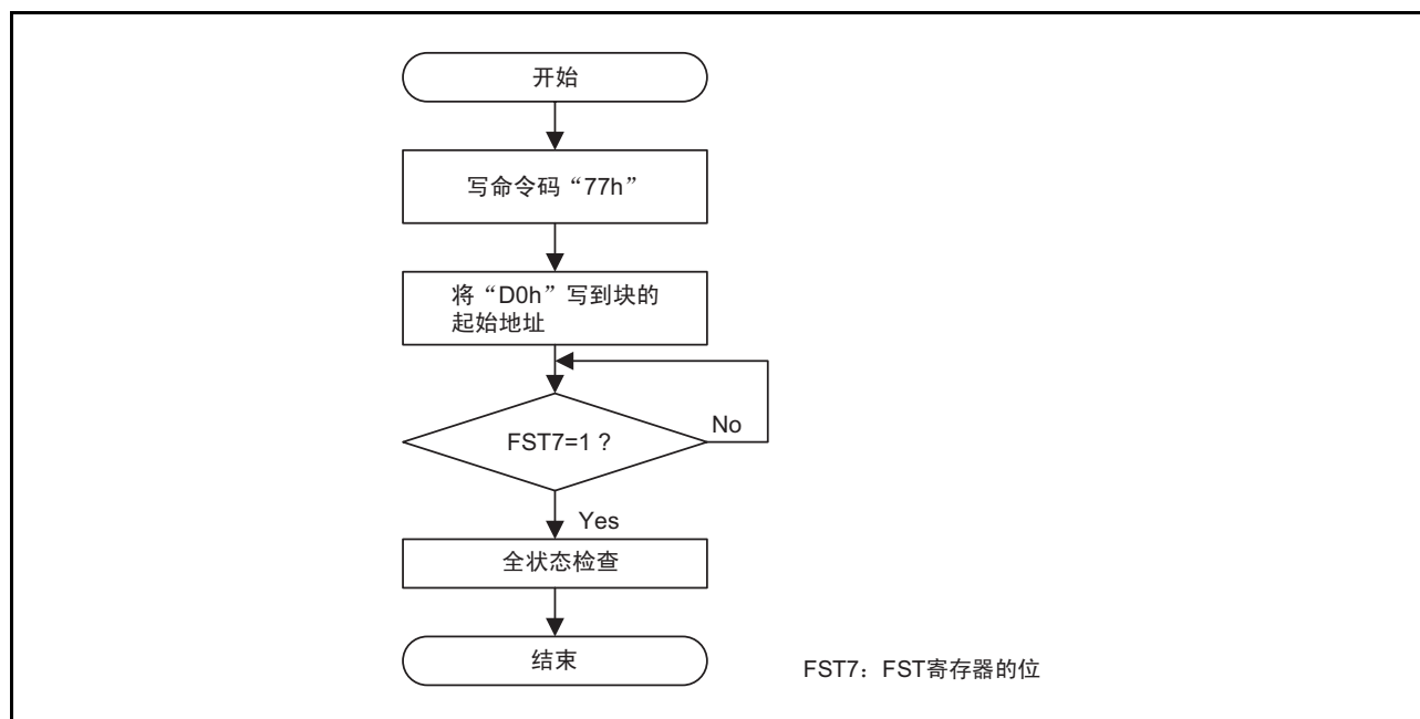
图 32.13 锁定位编程的流程图
