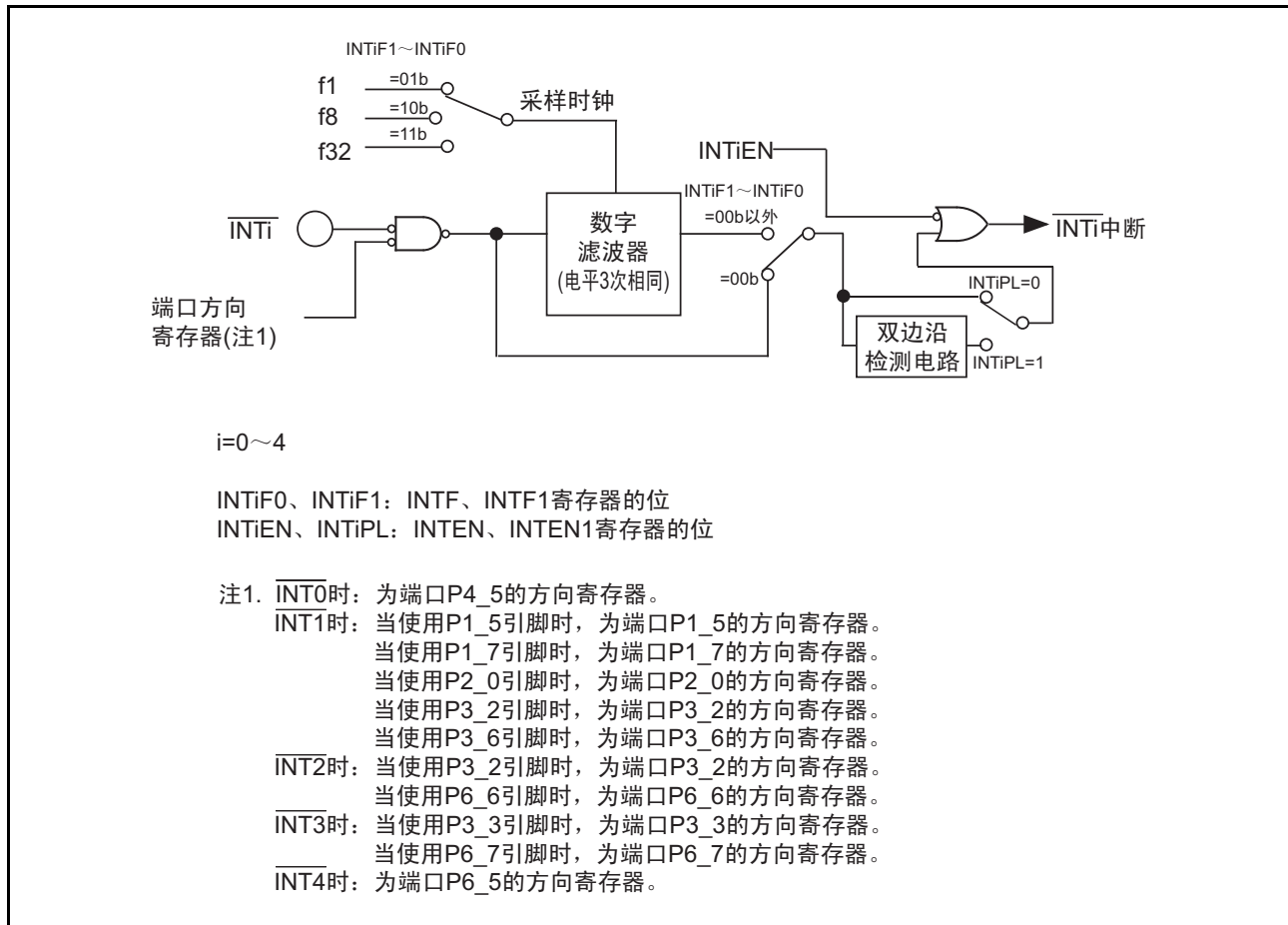
图 11.9 \overline{\text{INTi}} 输入滤波器的结构
