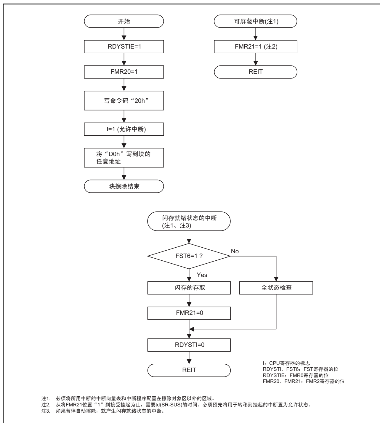
图 32.12 块擦除的流程图（允许闪存就绪状态的中断和挂起）
