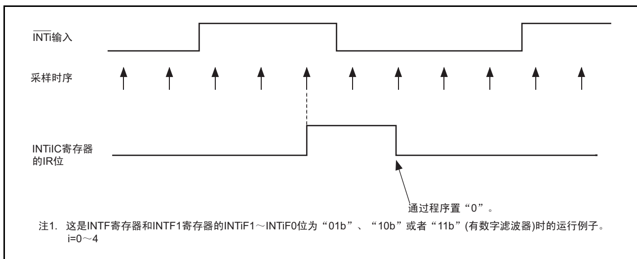
图 11.10 \overline{\text{INTi}} 输入滤波器的运行例子
