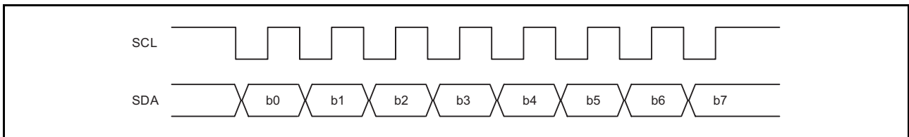
图 26.13 时钟同步串行格式的传送格式
