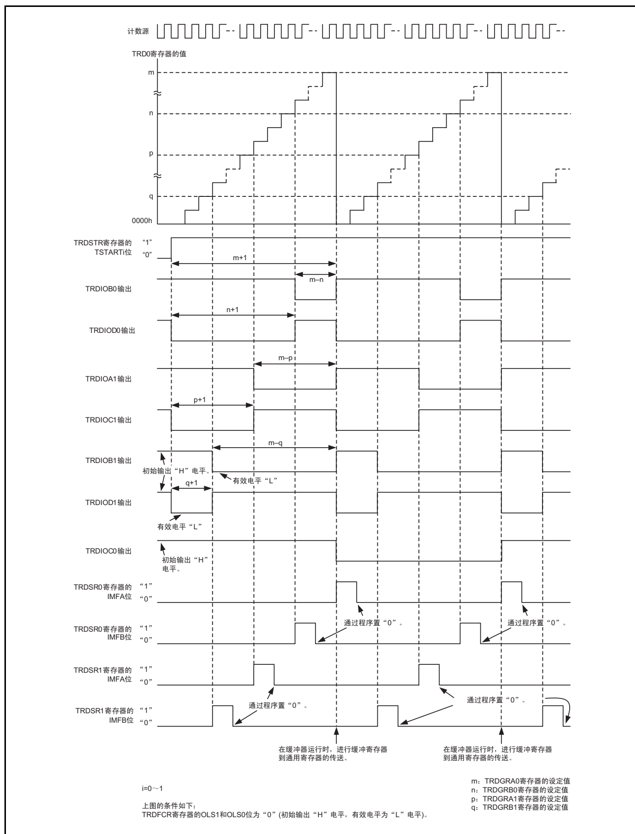
图 20.18 复位同步 PWM 模式的运行例子
