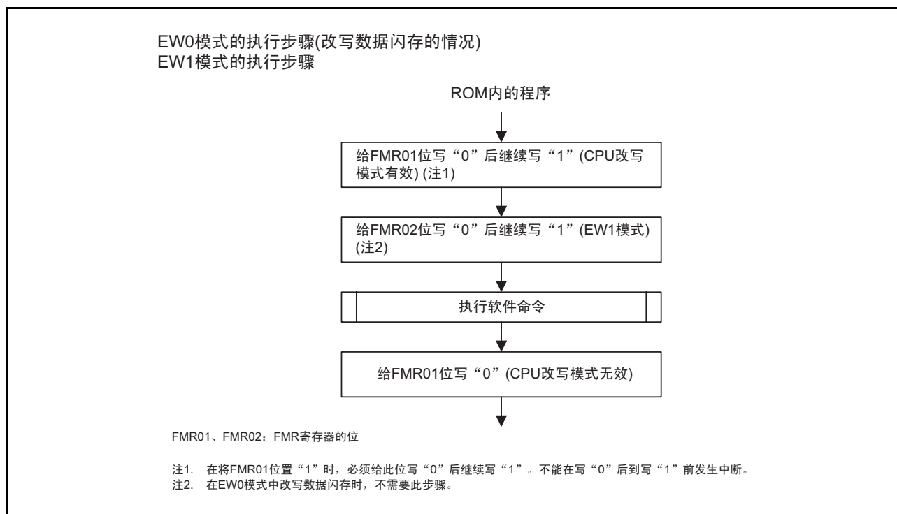
图 32.5 EW0 模式（改写数据闪存的情况）和 EW1 模式的设定和解除方法
