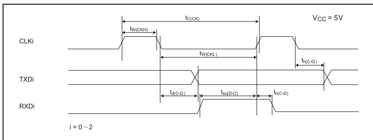
图 34.10 V_{CC}=5V 时的串行接口时序
