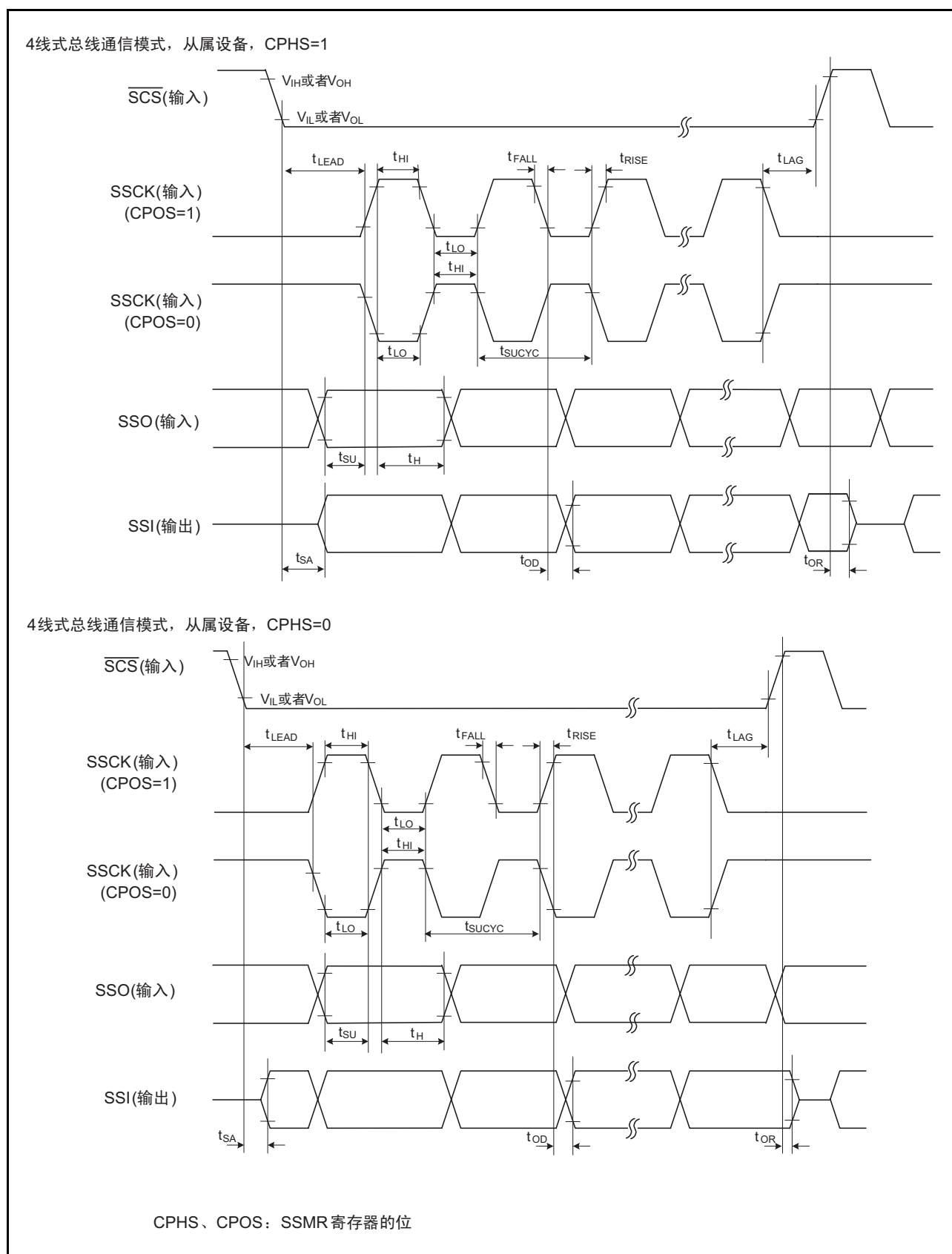
图 34.5 带片选的时钟同步串行 I/O 的输入 / 输出时序（从属器件）
