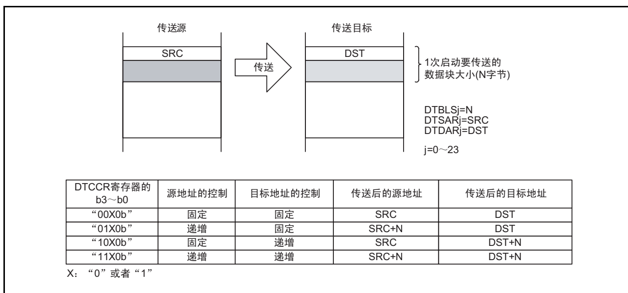
图 15.8 正常模式的数据传送
