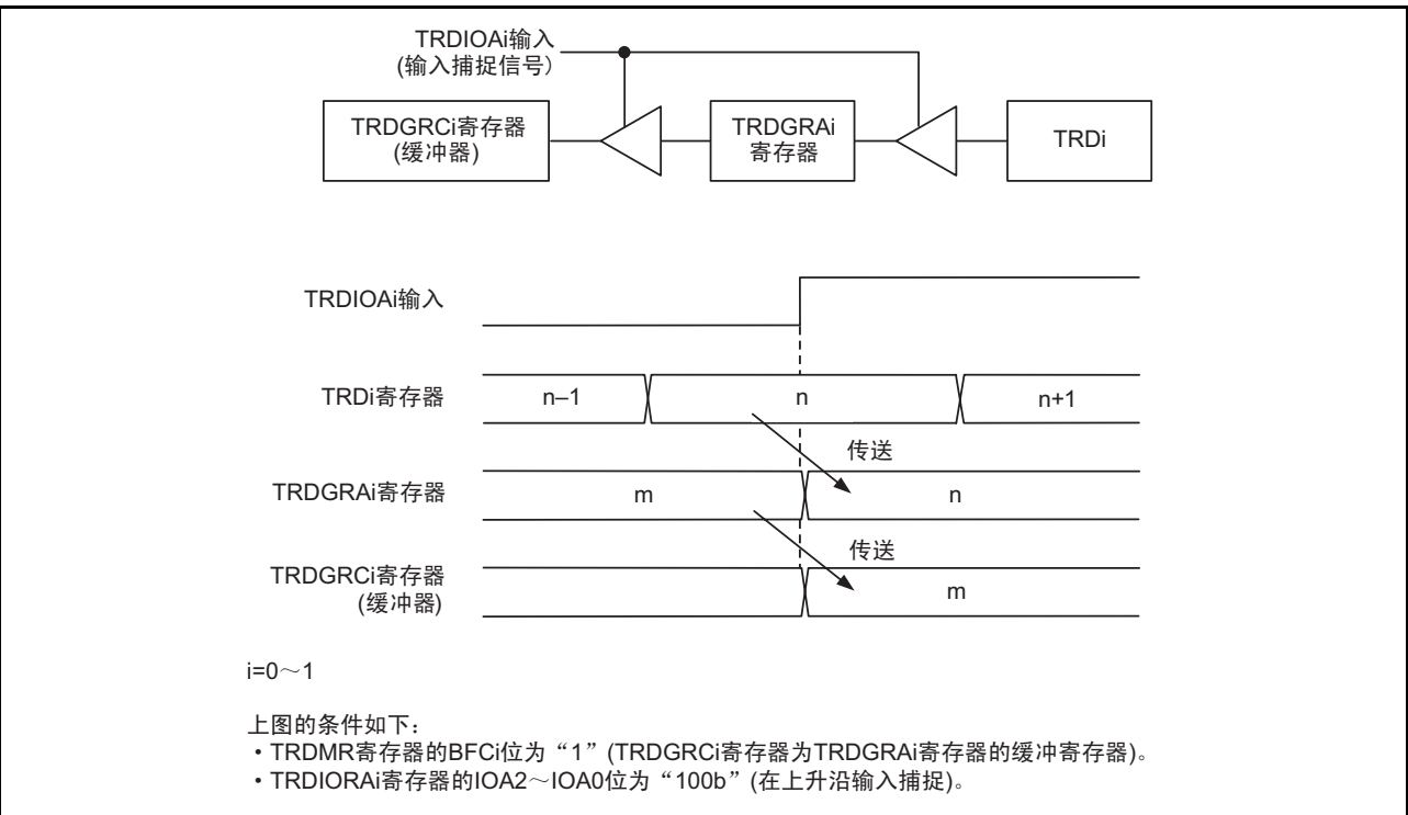
图 20.3 输入捕捉功能的缓冲器运行
