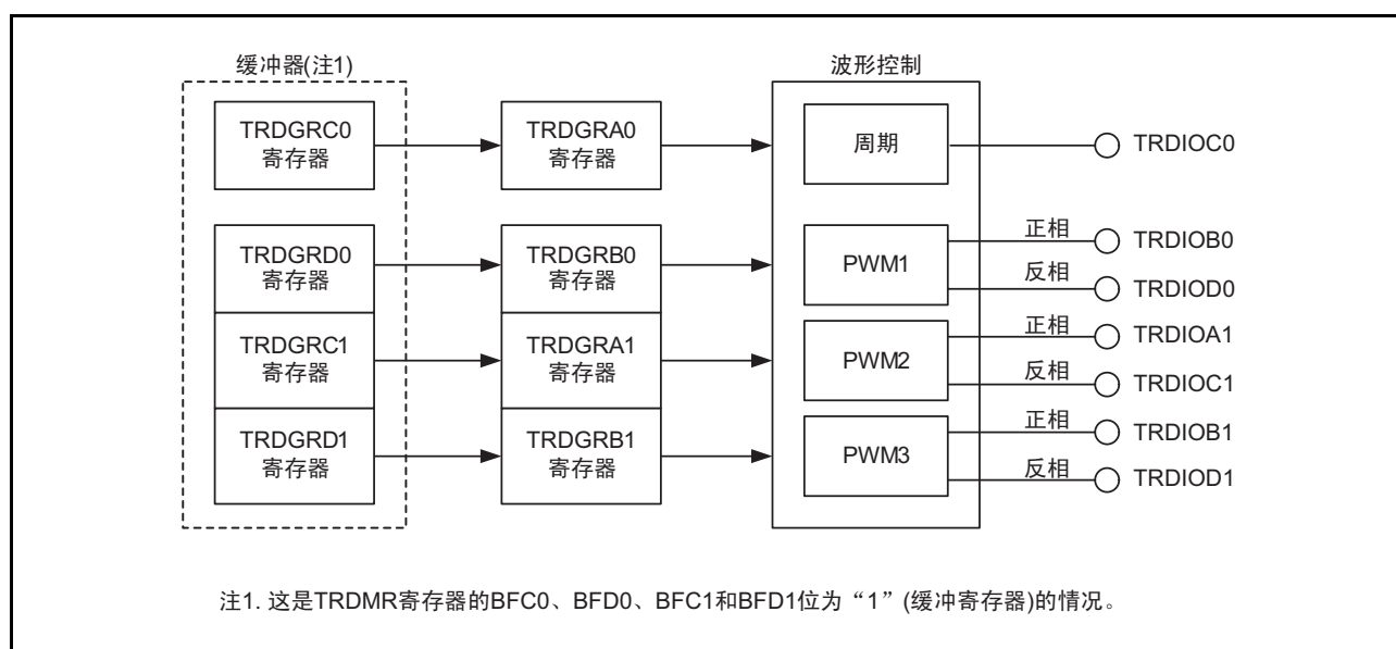
图 20.17 复位同步 PWM 模式的框图
