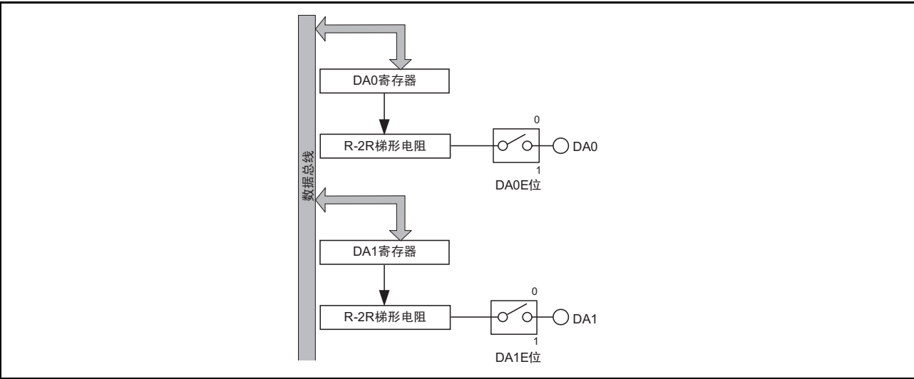
图 29.1 D/A 转换器的框图
