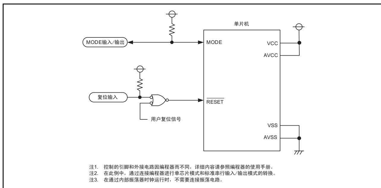
图 32.18 使用标准串行输入 / 输出模式 3 时的引脚处理例子
