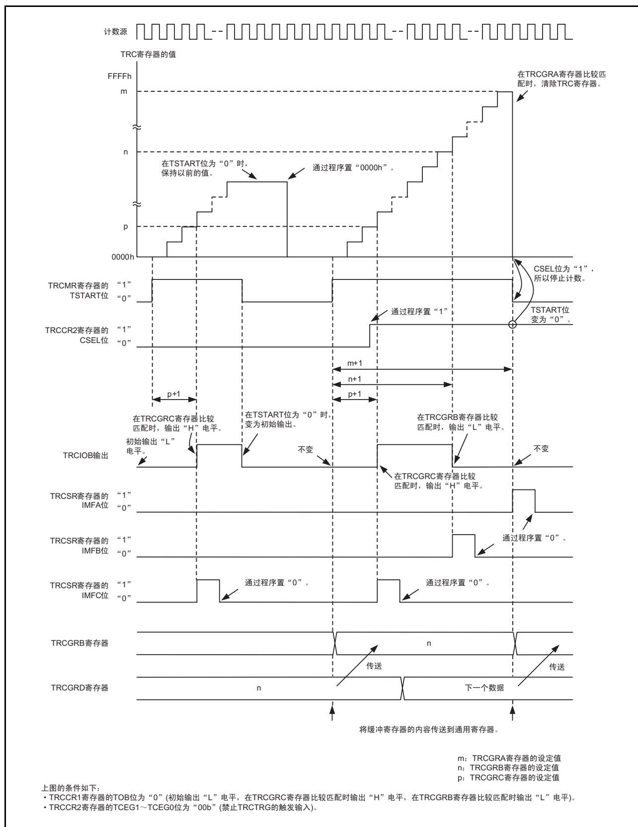
图 19.17 PWM2 模式的运行例子（禁止 TRCTRГ 触发输入）
