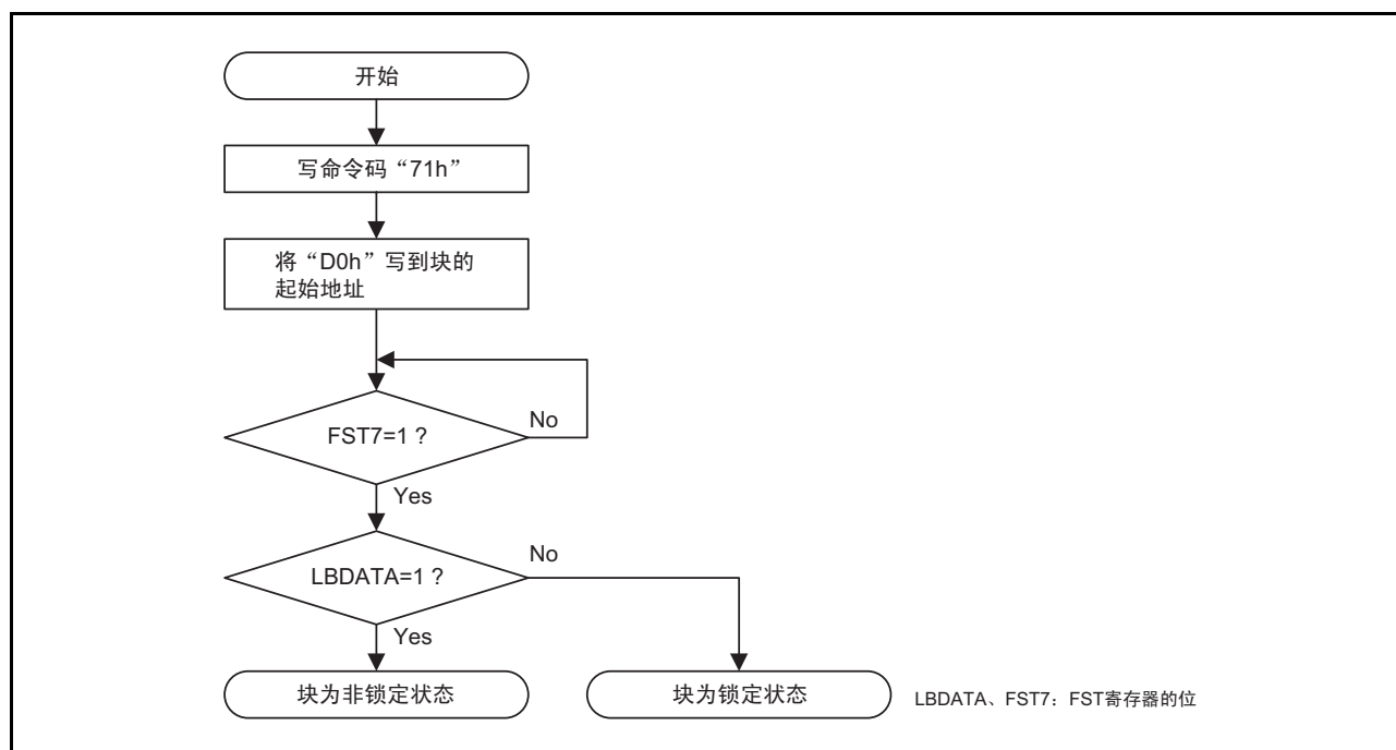
图 32.14 读锁定位状态的流程图
