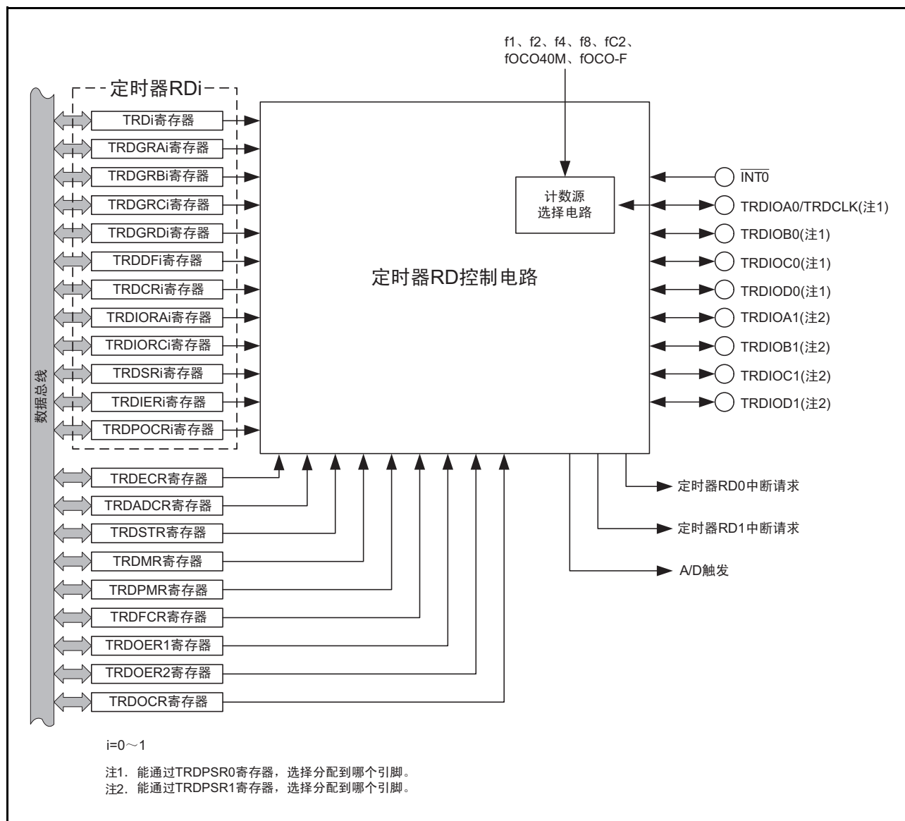
图 20.1 定时器 RD 的框图
