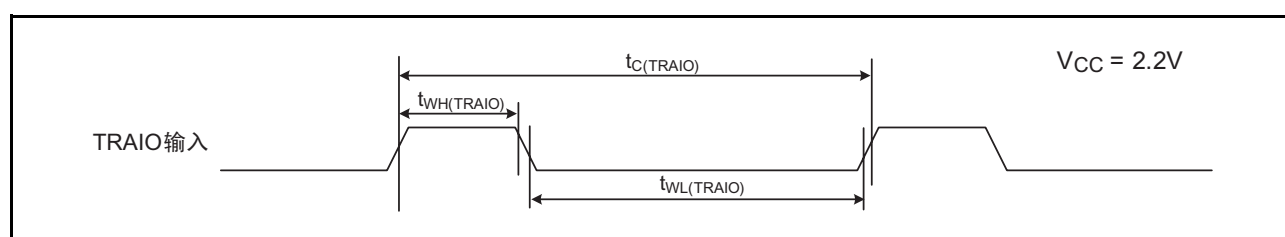
图 34.17 V_{CC}=2.2V 时的 TRAIO 输入时序
