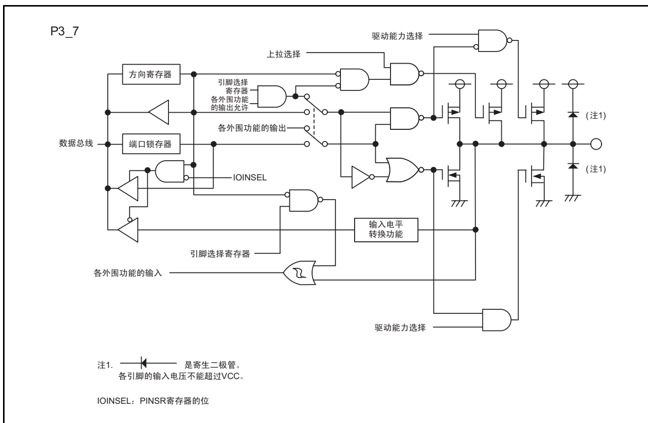
图 7.9 I/O 端口的结构 (9)
