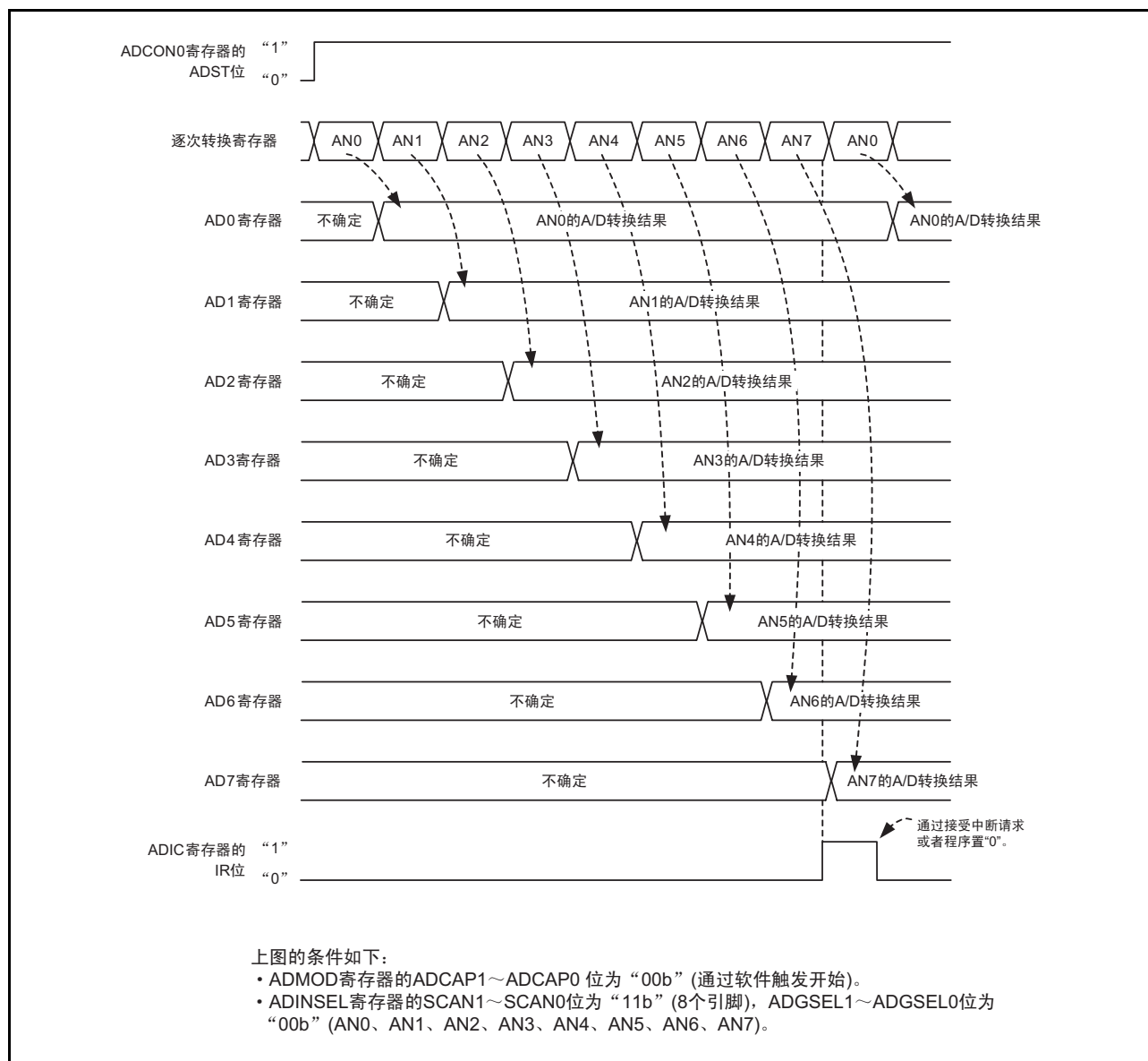
图 28.9 重复扫描模式的运行例子
