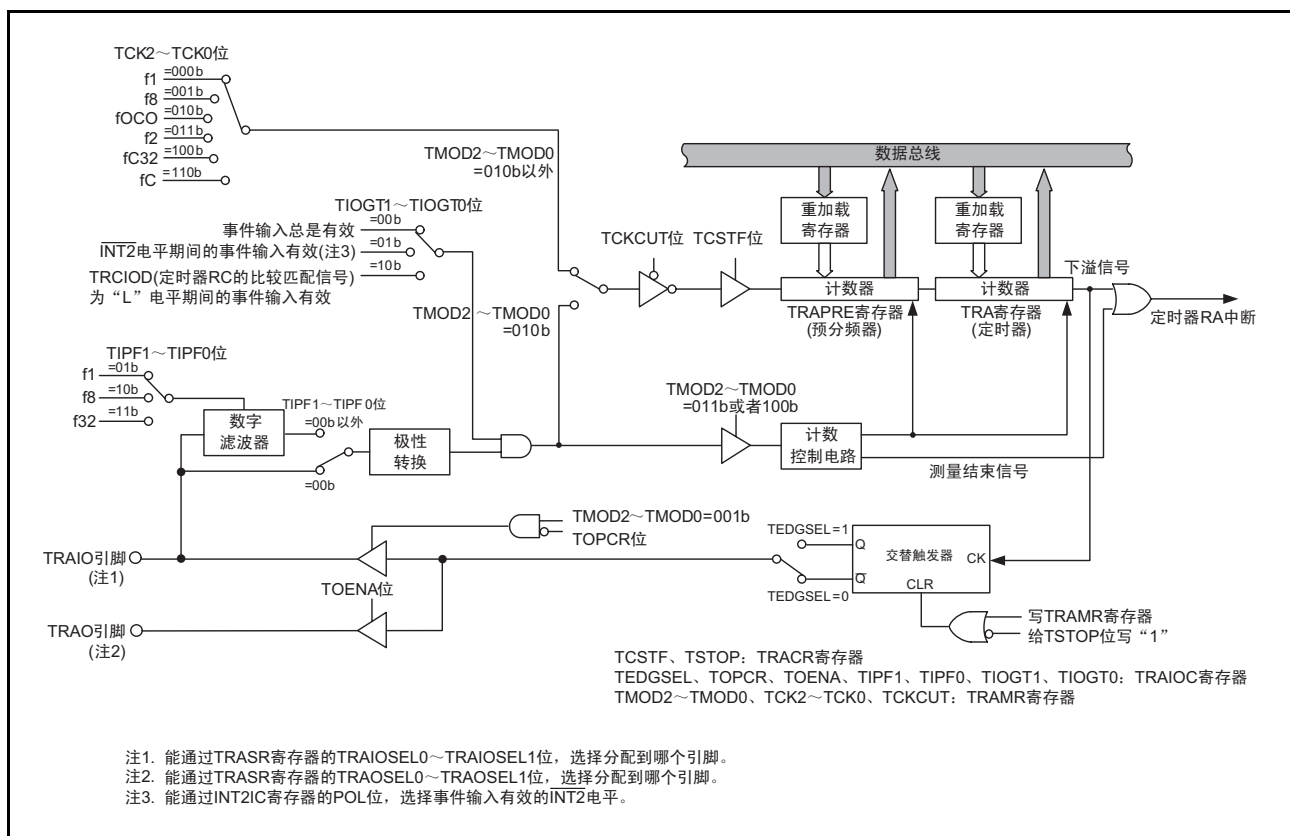
图 17.1 定时器 RA 的框图
