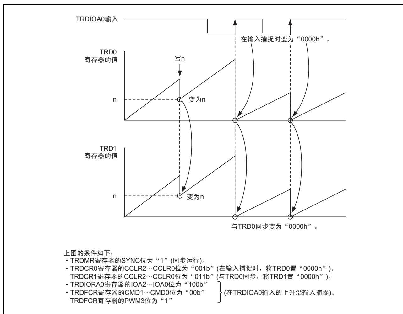
图 20.5 同步运行
