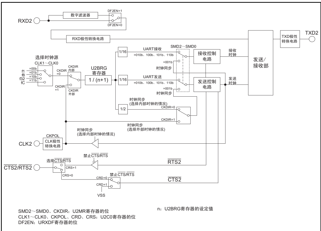
图 23.1 UART2 的框图
