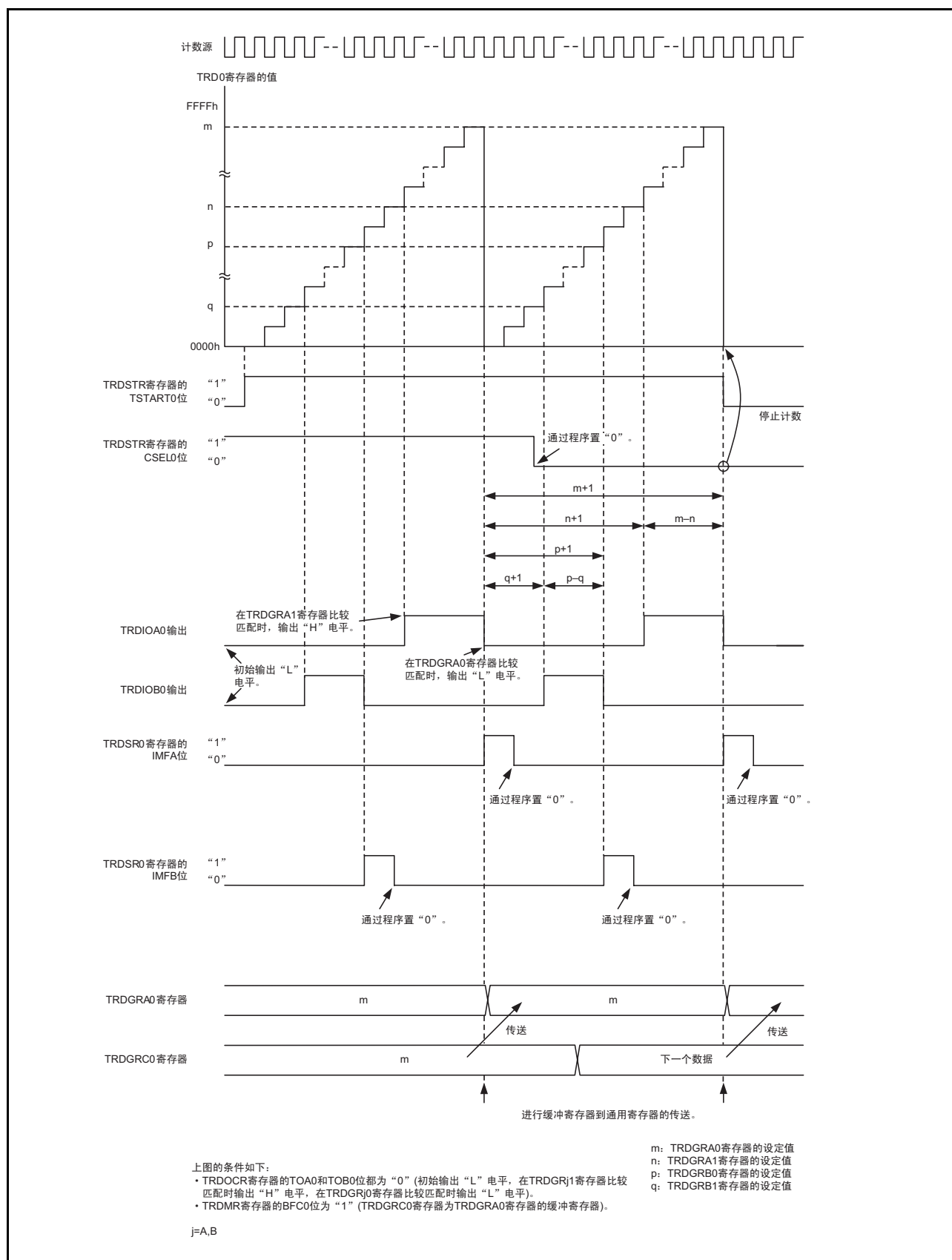
图 20.23 PWM3 模式的运行例子
