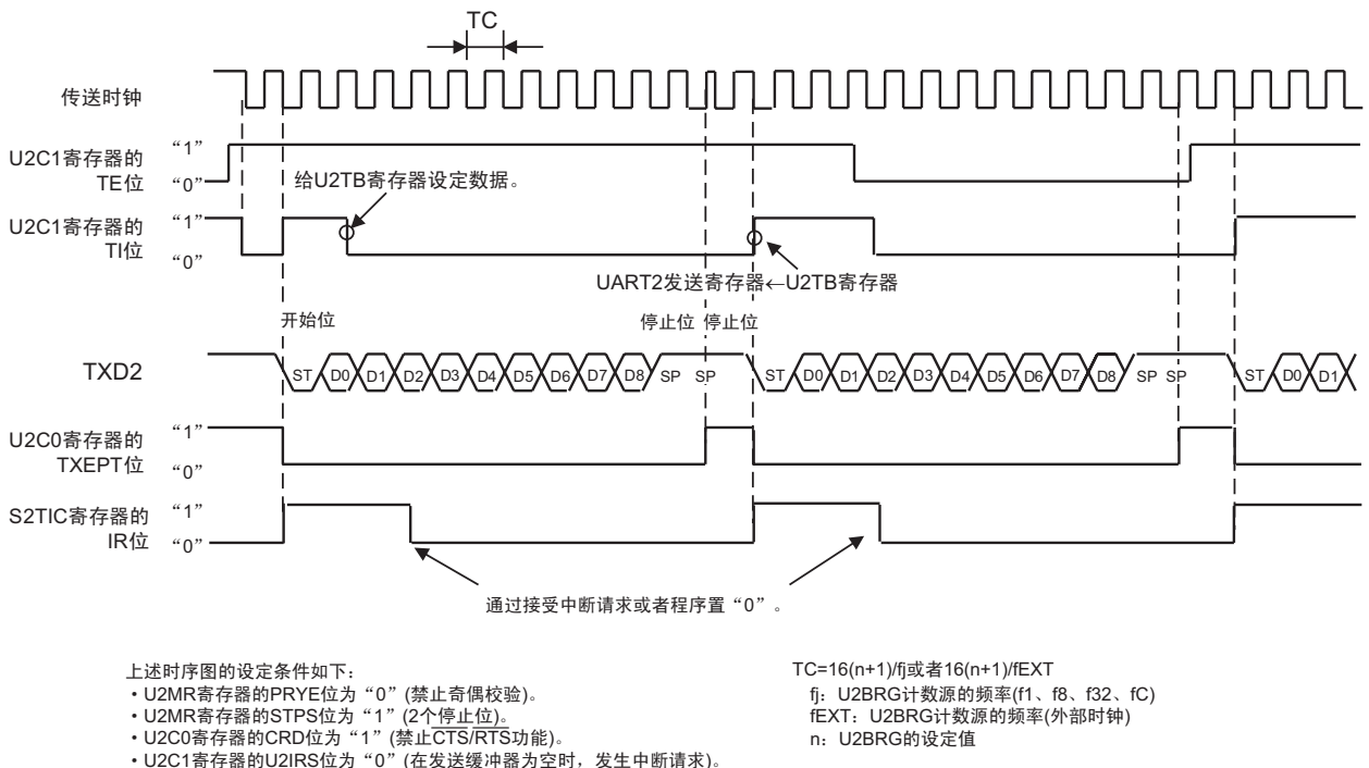
图 23.7 UART 模式的发送时序例子
