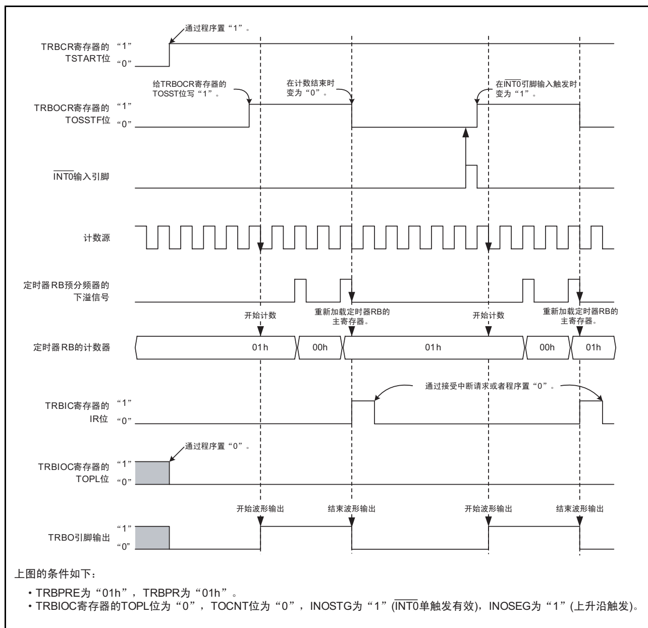
图 18.4 可编程单触发生模式的运行例子
