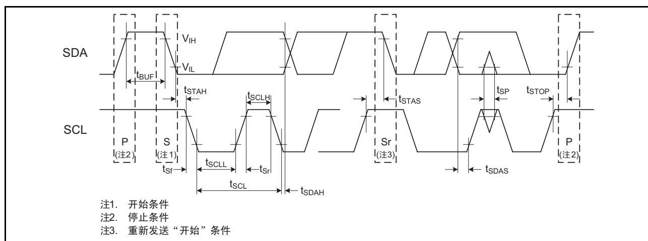
图 34.7 I²C 总线接口的输入 / 输出时序
