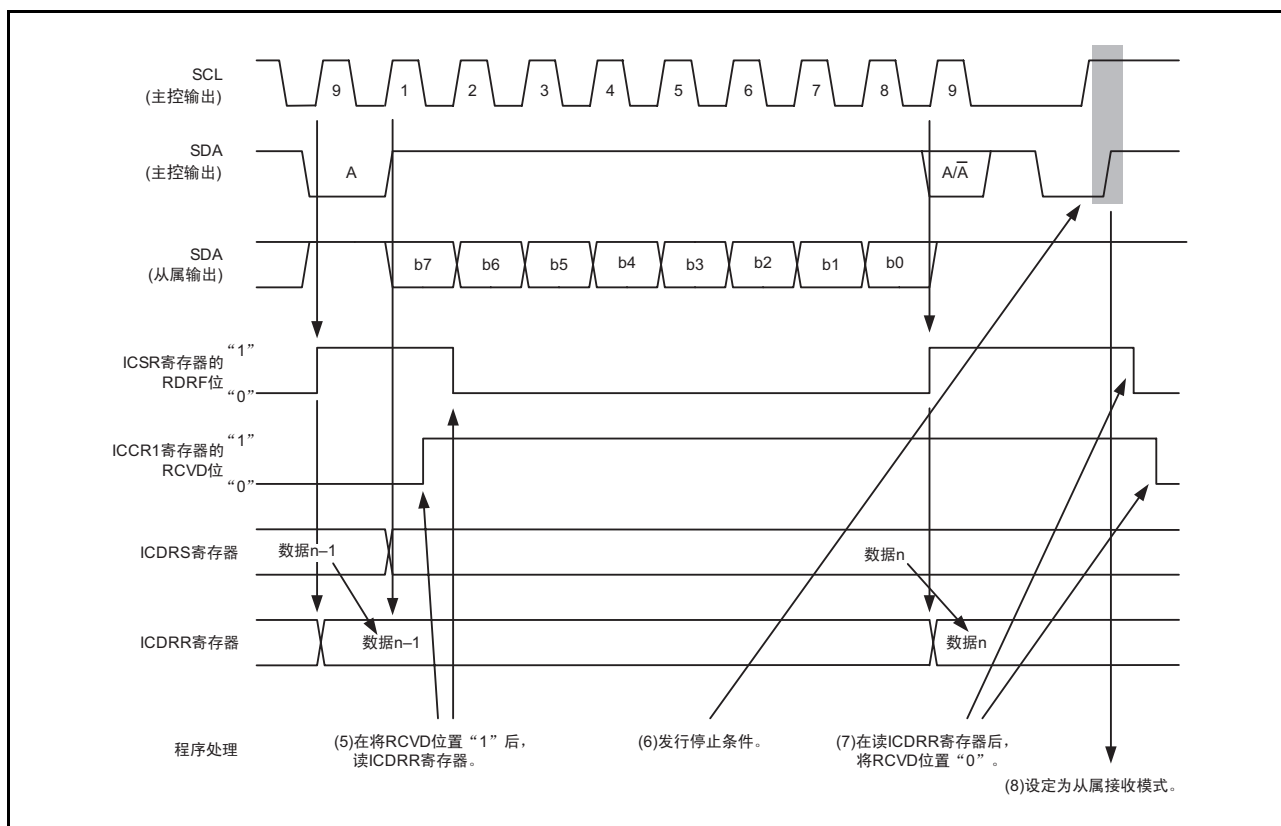
图 26.8 主控接收模式的运行时序（I 2 C 总线接口模式）（2）
