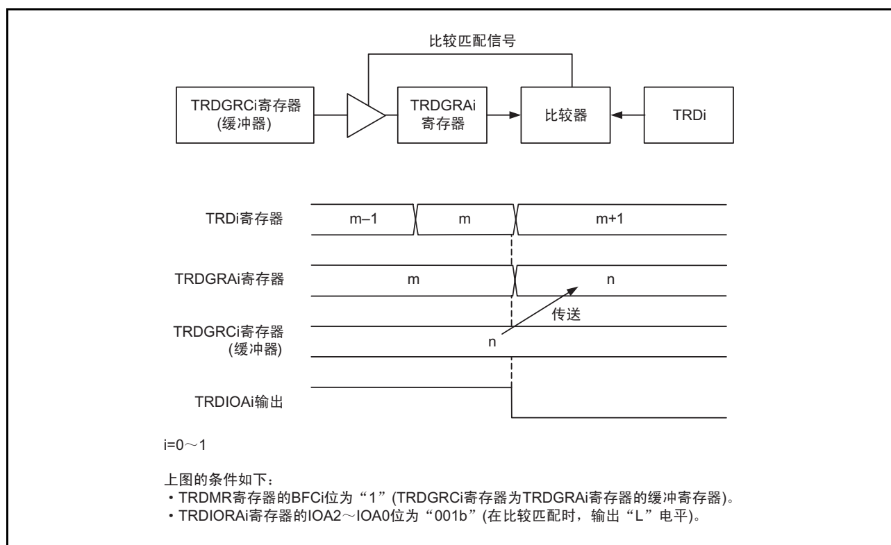
图 20.4 输出比较功能的缓冲器运行
