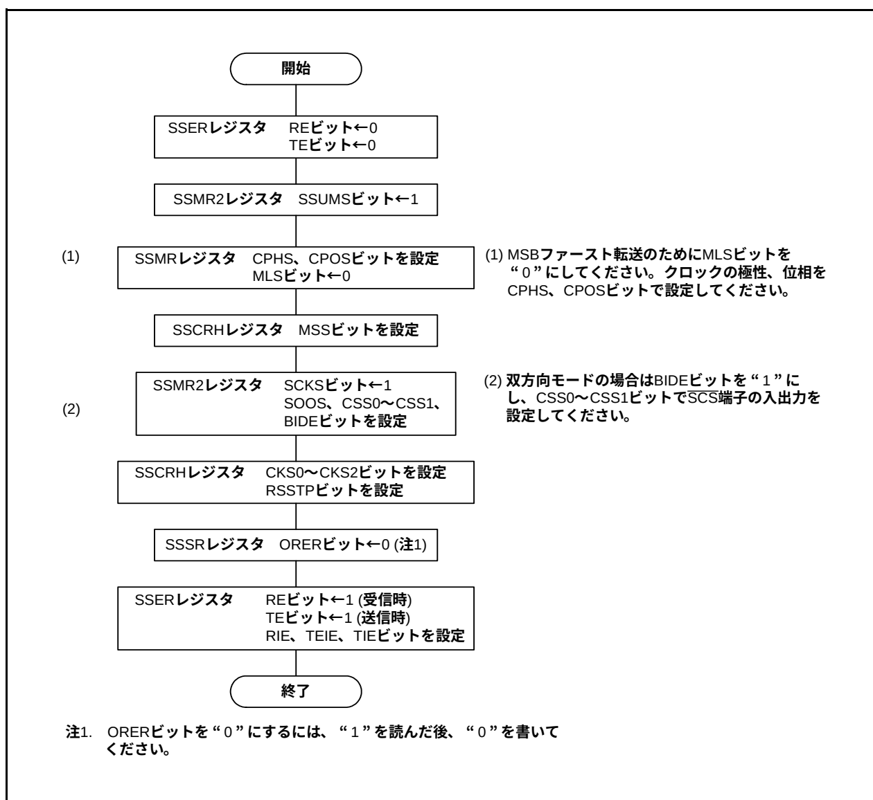
図16.18 4線式バス通信モードの初期化
