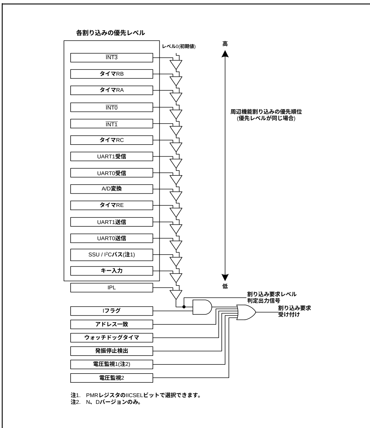
図12.11 割り込み優先レベルの判定回路
