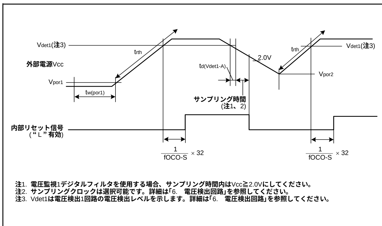
図 20.22 パワーオンリセット回路の電氣的特性
