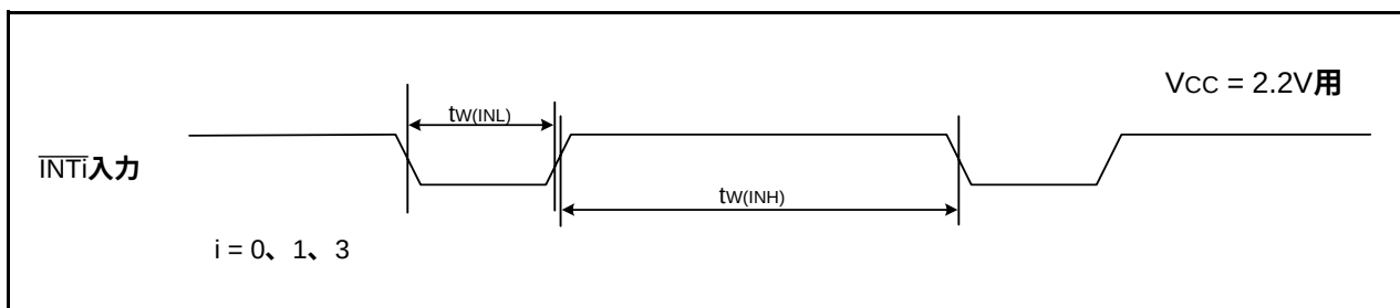
図 20.19 Vcc = 2.2V時の外部割り込み \overline{INTi} 入力タイミング
