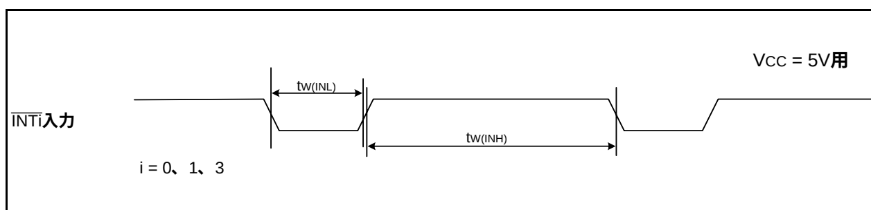
図 20.30 Vcc = 5V時の外部割り込み \overline{INTi} 入力タイミング
