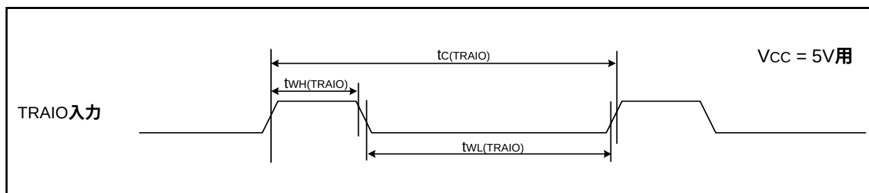
図20.28 V_{CC} = 5V 時のTRAIO入力タイミング
