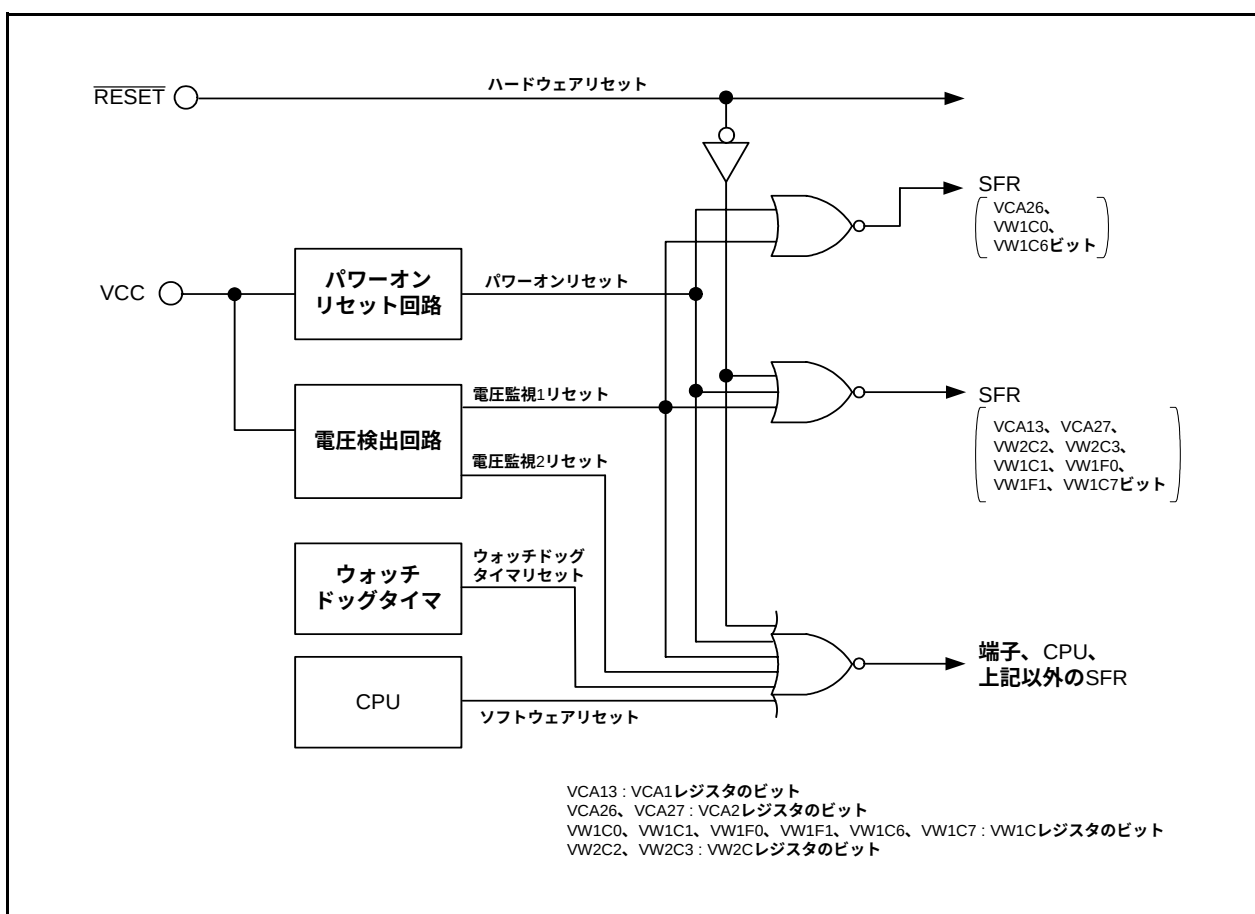
図5.2 リセット回路のブロック図(J、Kバージョン)
