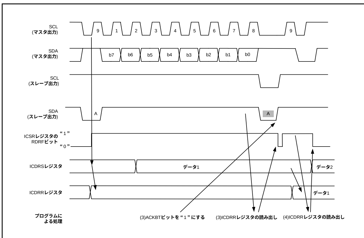
図 16.39 スレーブ受信モードの動作タイミング (I²C バスインタフェースモード) (2)
