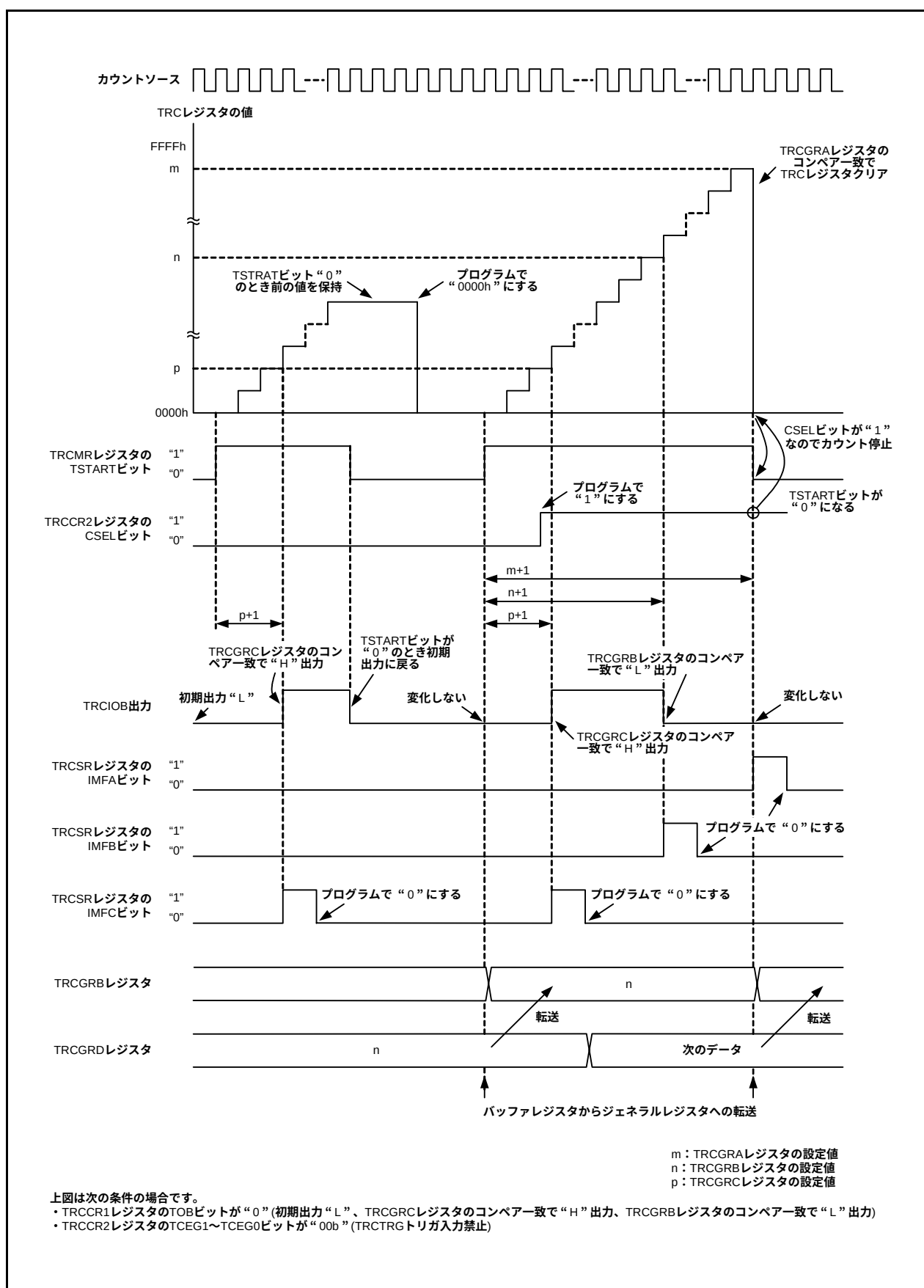
図14.57 PWM2モードの動作例 (TRCTRГ トリガ入力禁止の場合)
