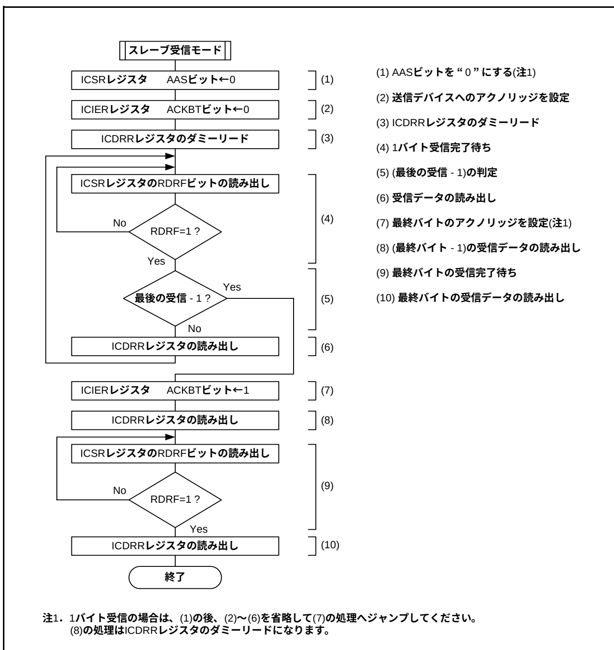
図 16.48 スレープ受信モードのレジスタ設定例(I²Cバスインタフェースモード)
