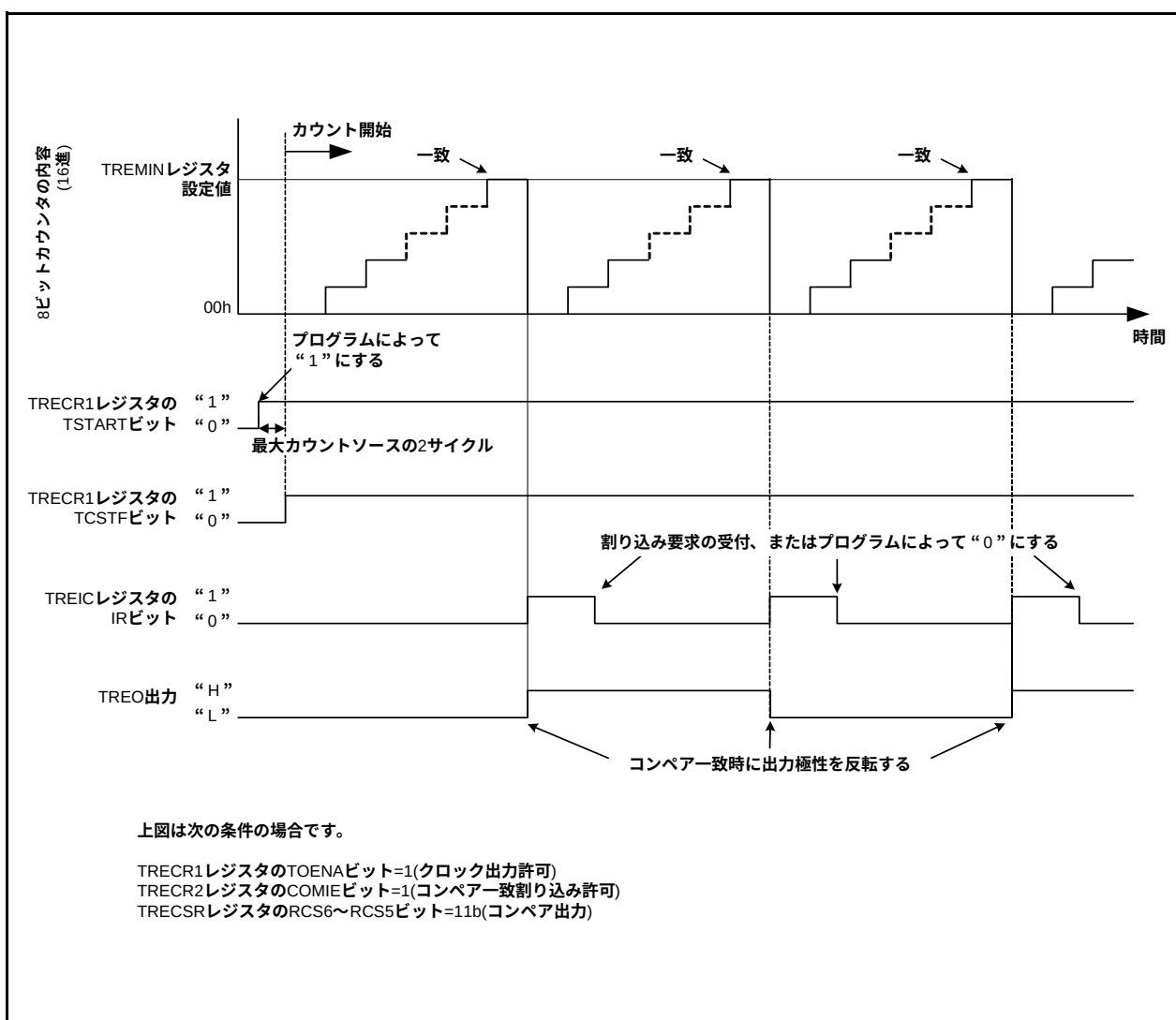
図 14.77 アウトプットコンペアモードの動作例
