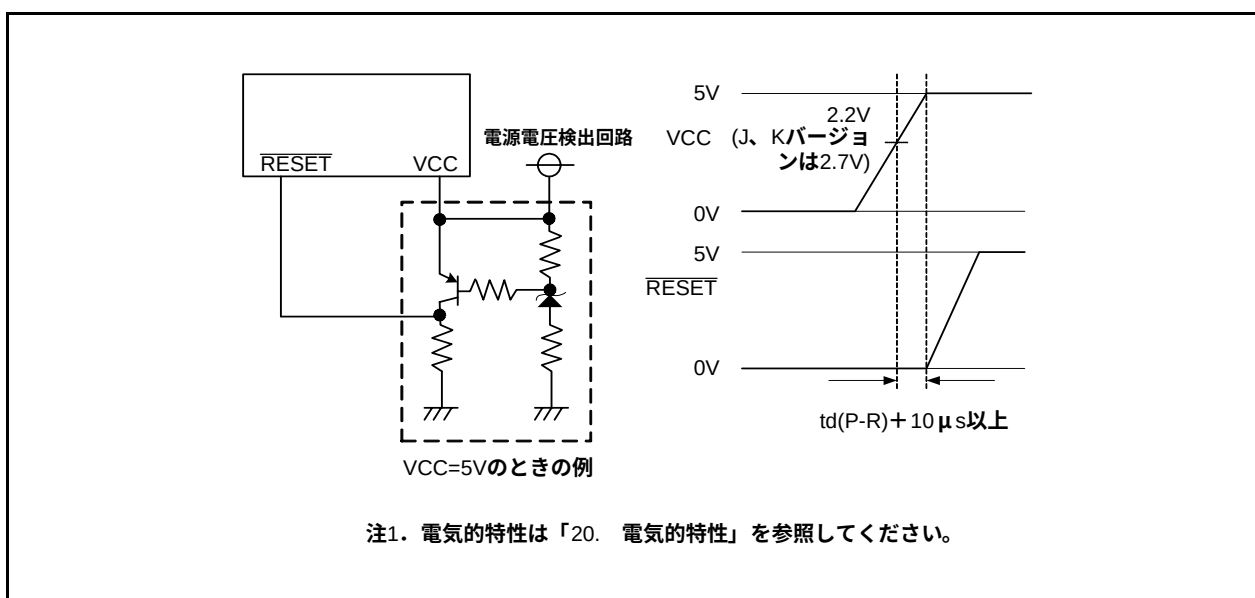
図5.7 ハードウェアリセット回路例(外付け電源電圧検出回路の使用例)と動作
