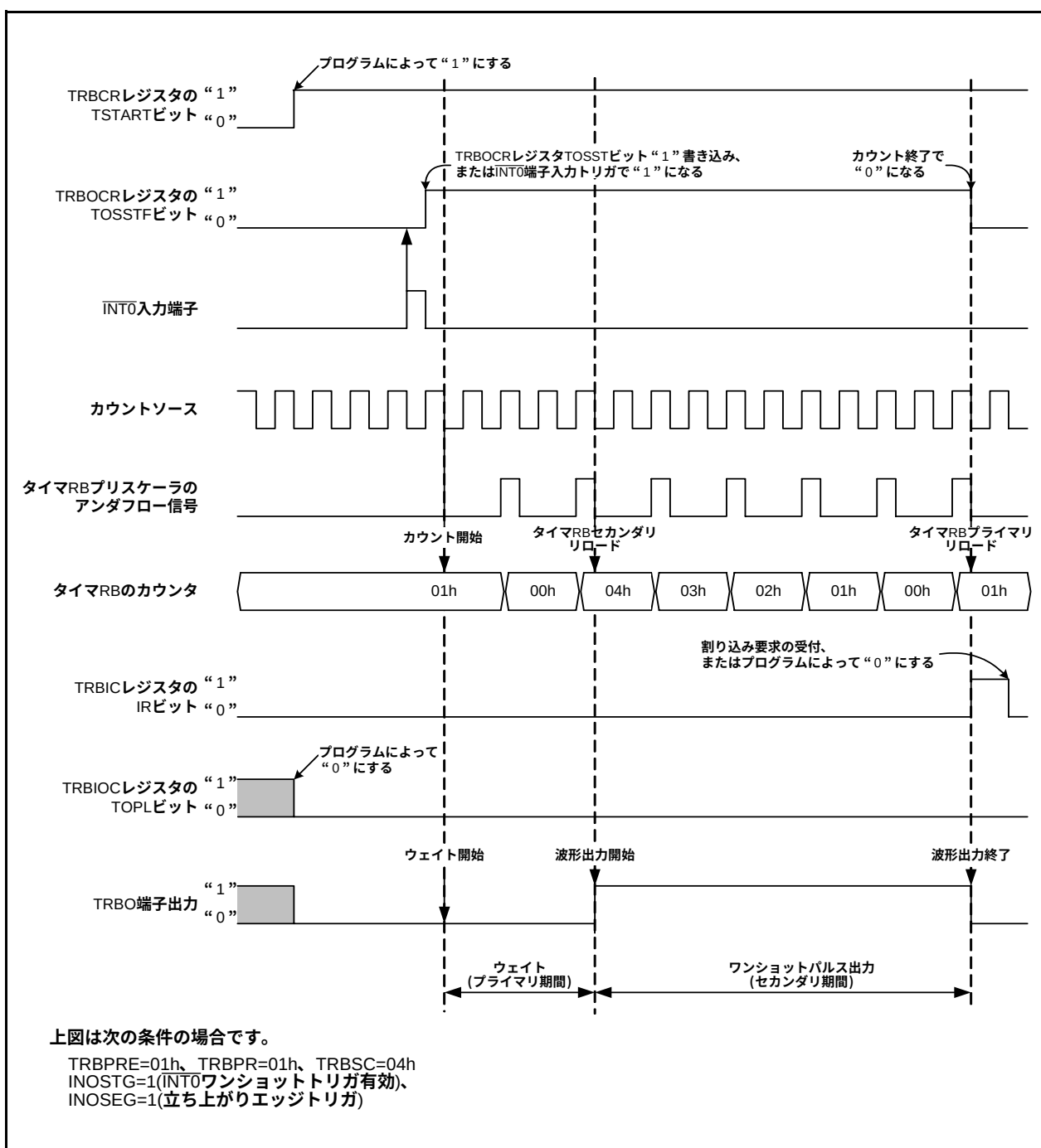
図14.23 プログラマブルウェイトワンショット発生モードの動作例
