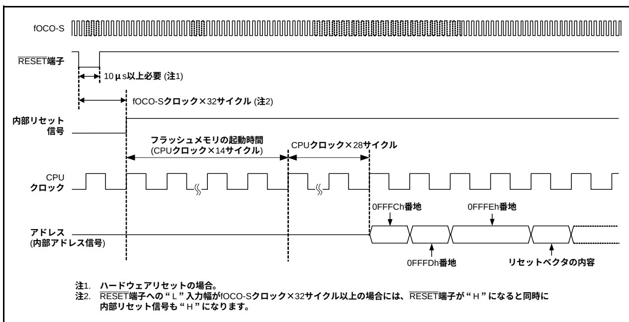
図5.4 リセットシーケンス
