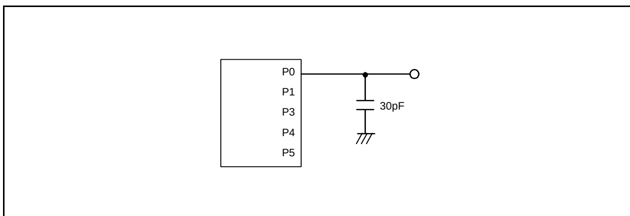
図 20.1 ポート P0、P1、P3 ~ P5 のタイミング測定回路
