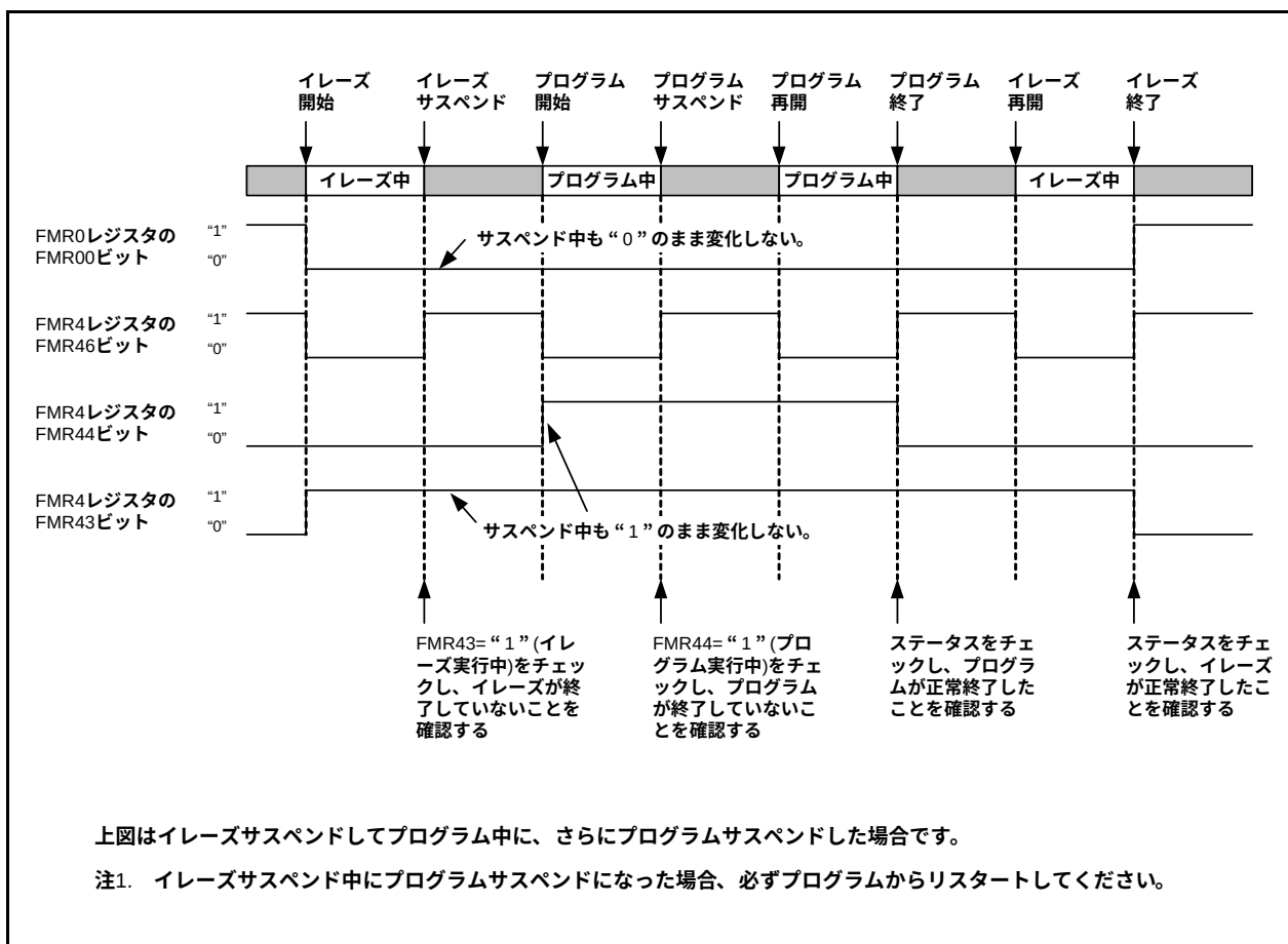
図19.8 サスペンド動作に関するタイミング
