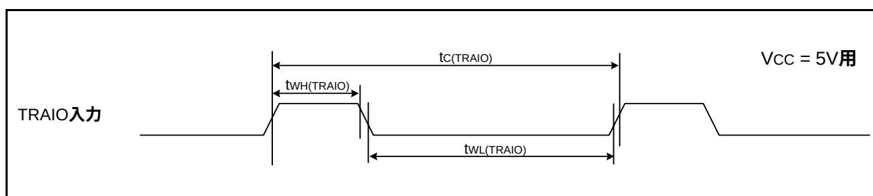
図20.9 V_{CC} = 5V 時のTRAIO入力タイミング
