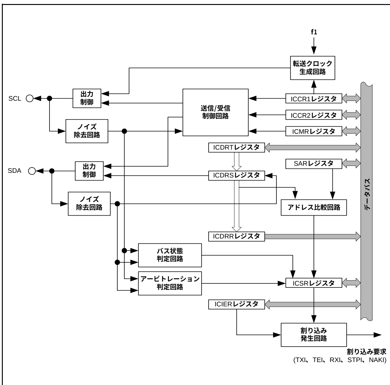
図 16.22 I 2 C バスインタフェースブロック図
