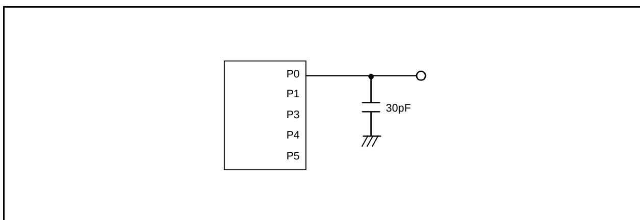
図 20.20 ポート P0、P1、P3～P5 のタイミング測定回路
