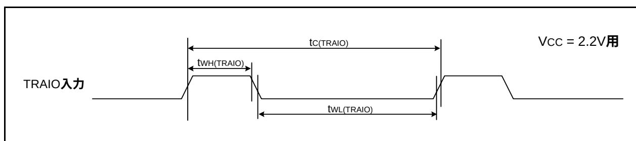
図20.17 V_{CC} = 2.2V 時のTRAIO入力タイミング
