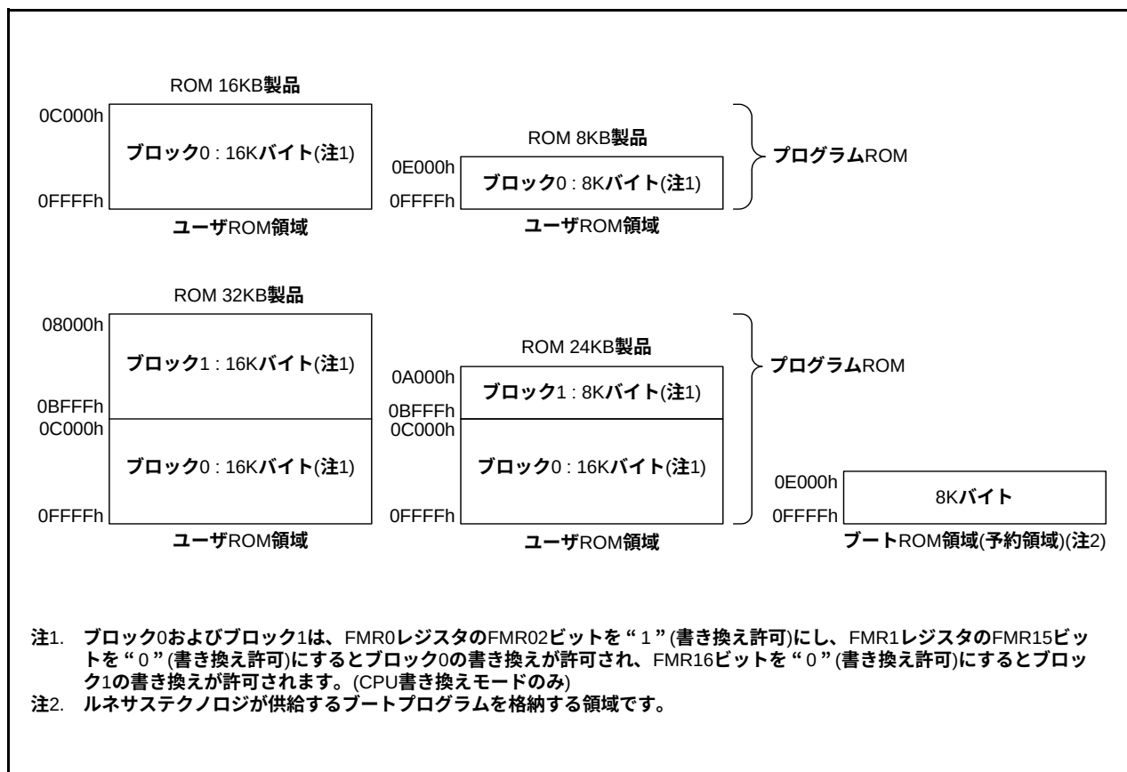
図19.1 R8C/26グループのフラッシュメモリのブロック図
