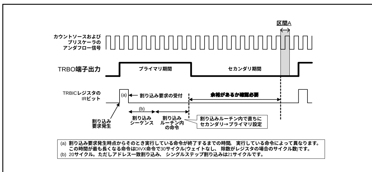
図14.24 対策例(a)のタイマRB割り込みを使用する例
