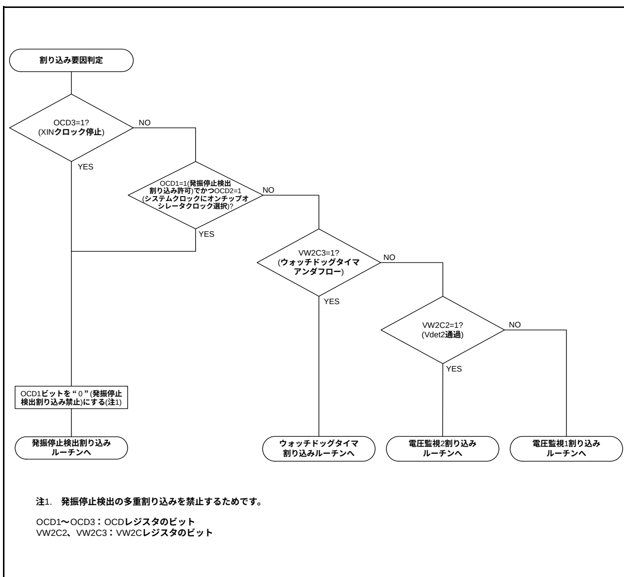
図 10.19 発振停止検出割り込み、ウォッチドッグタイマ割り込み、電圧監視1割り込みまたは電圧監視2割り込みの割り込み要因判別方法例(N、Dバージョン)
