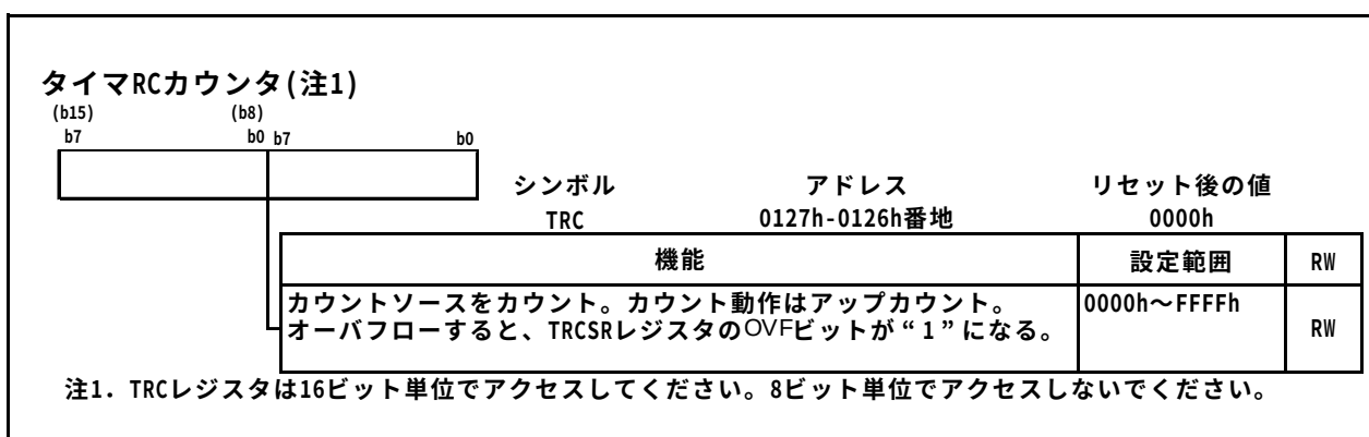
図14.31 TRCレジスタ
