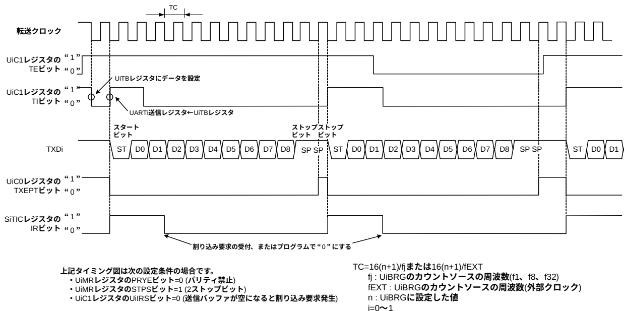
図 15.11 UART モード時の送信タイミング
