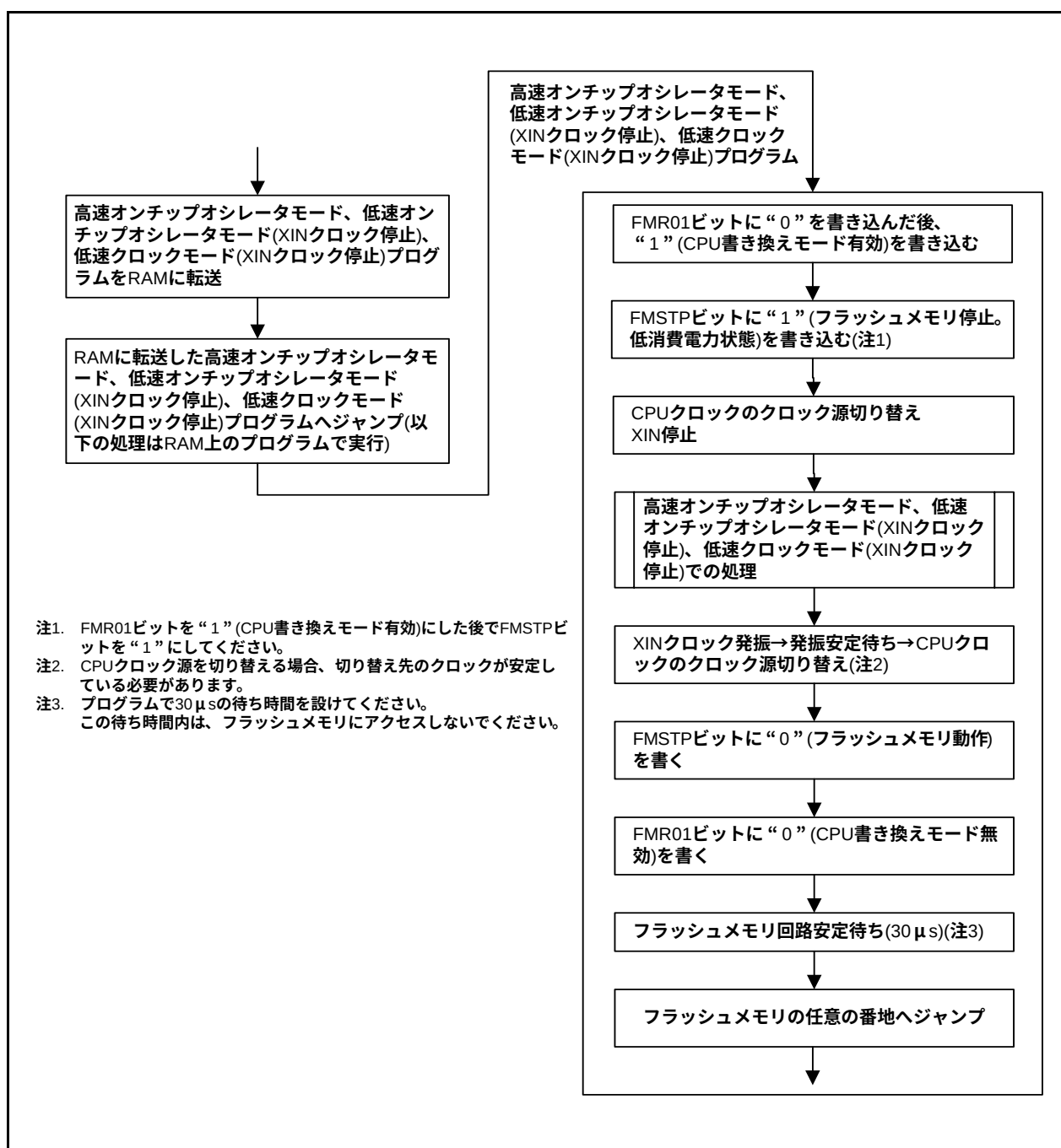
図 19.11 高速オンチップオシレータモード、低速オンチップオシレータモード(XINクロック停止)、低速クロックモード(XINクロック停止)でさらに低消費電力にする処理
