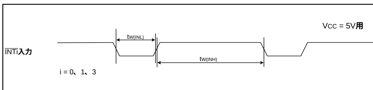
図 20.11 Vcc = 5V時の外部割り込み \overline{INTi} 入力タイミング
