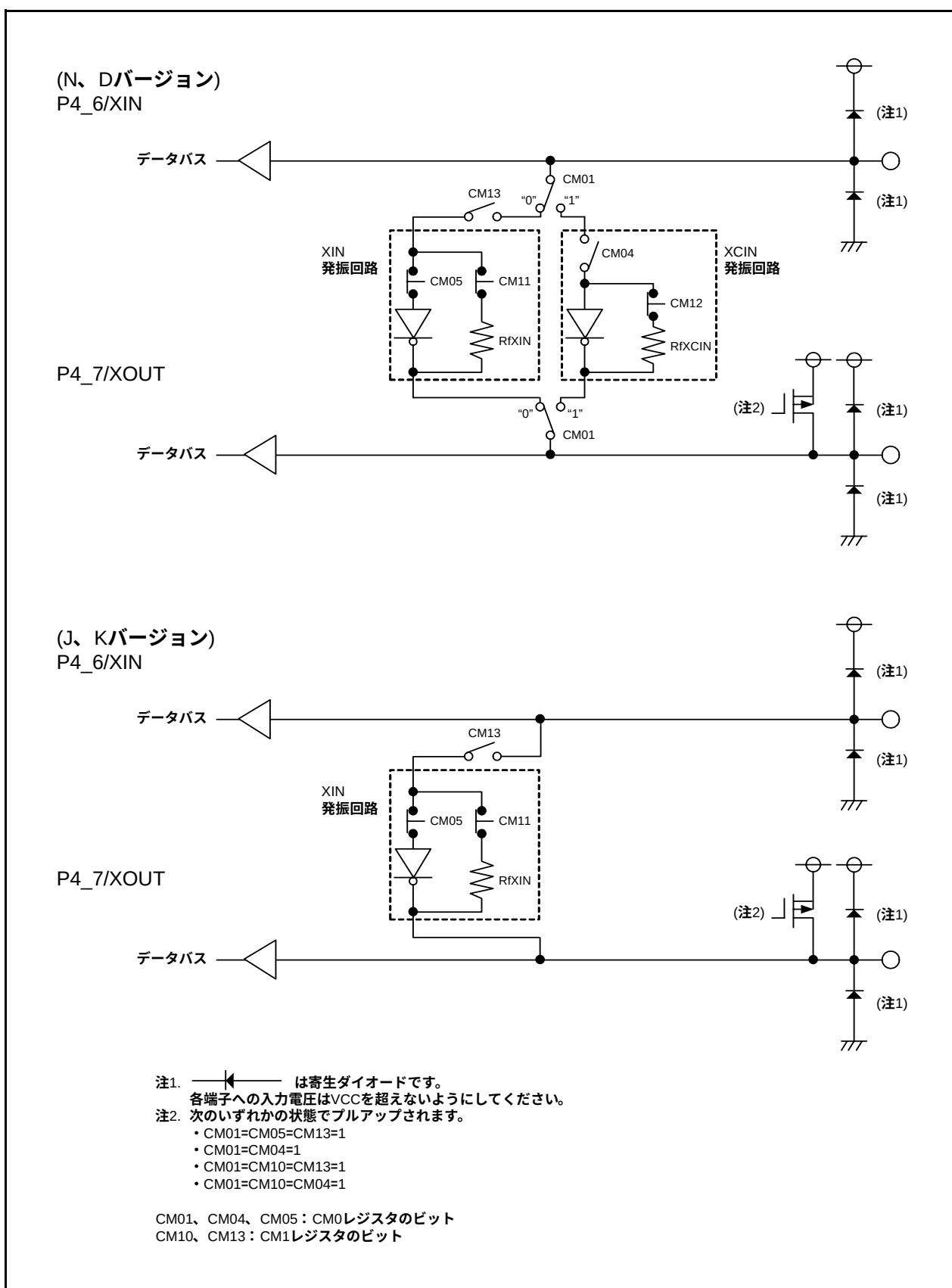
図7.5 プログラマブル入出力ポートの構成(5)
