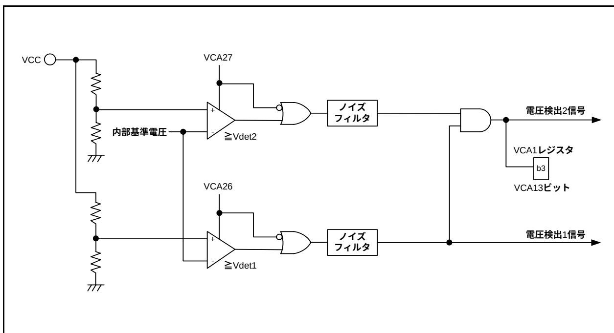
図6.2 電圧検出回路ブロック図(J、Kバージョン)
