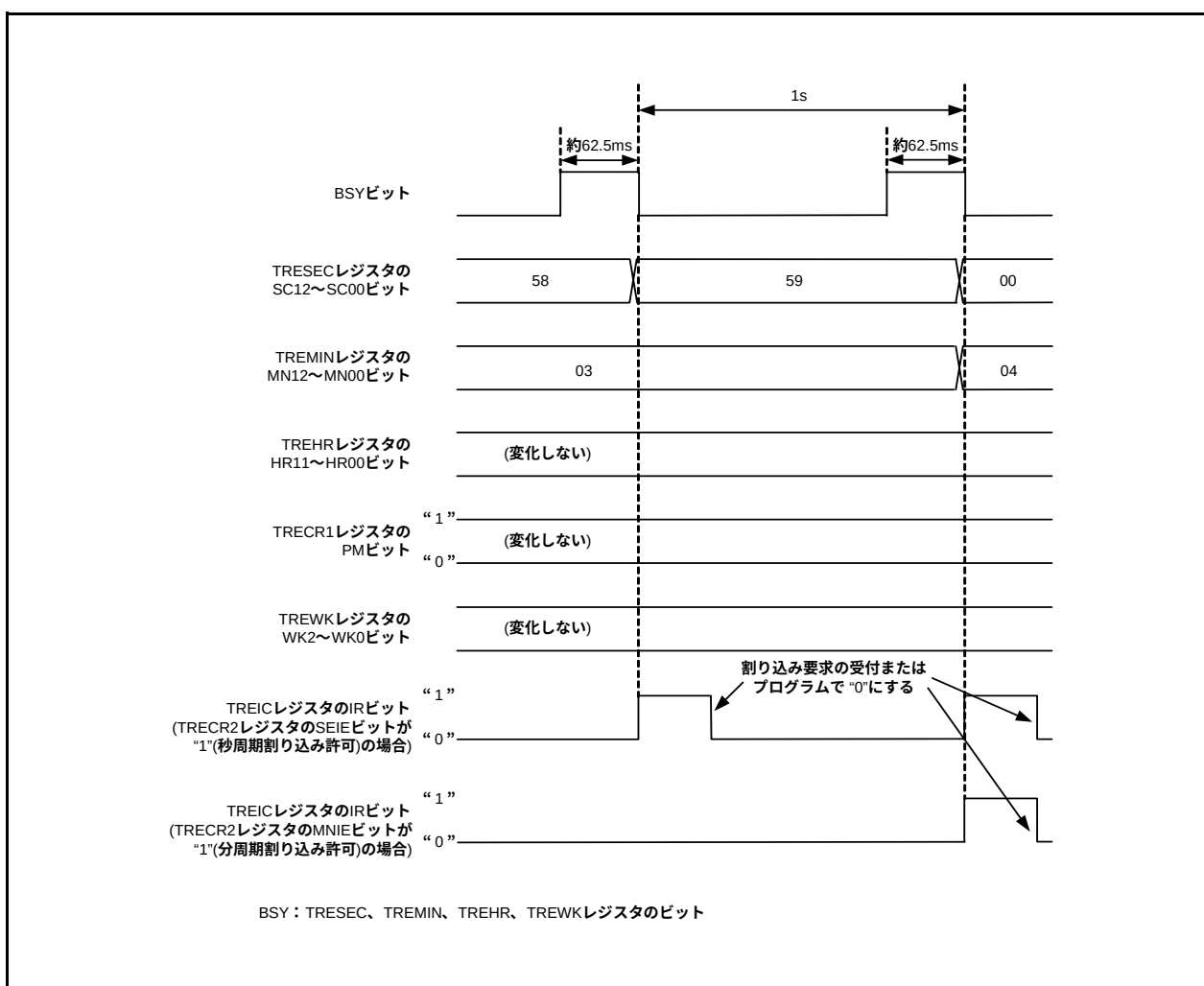
図 14.70 リアルタイムクロックモードの動作例
