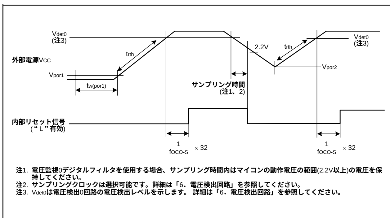
図 20.3 リセット回路の電気的特性
