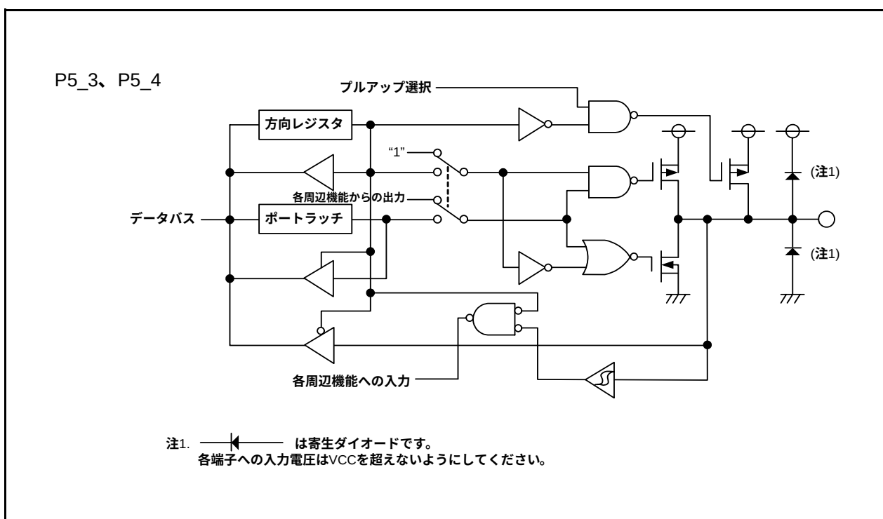
図 7.6 プログラマブル入出力ポートの構成 (6)
