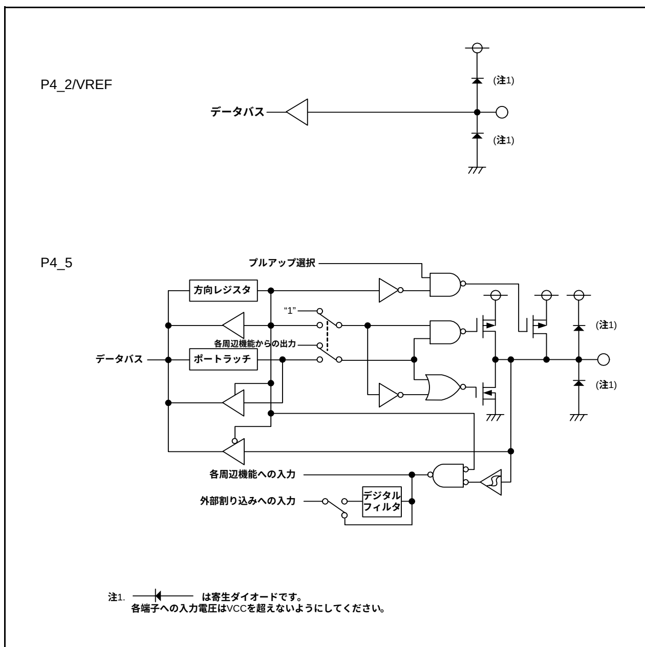
図7.4 プログラマブル入出力ポートの構成(4)
