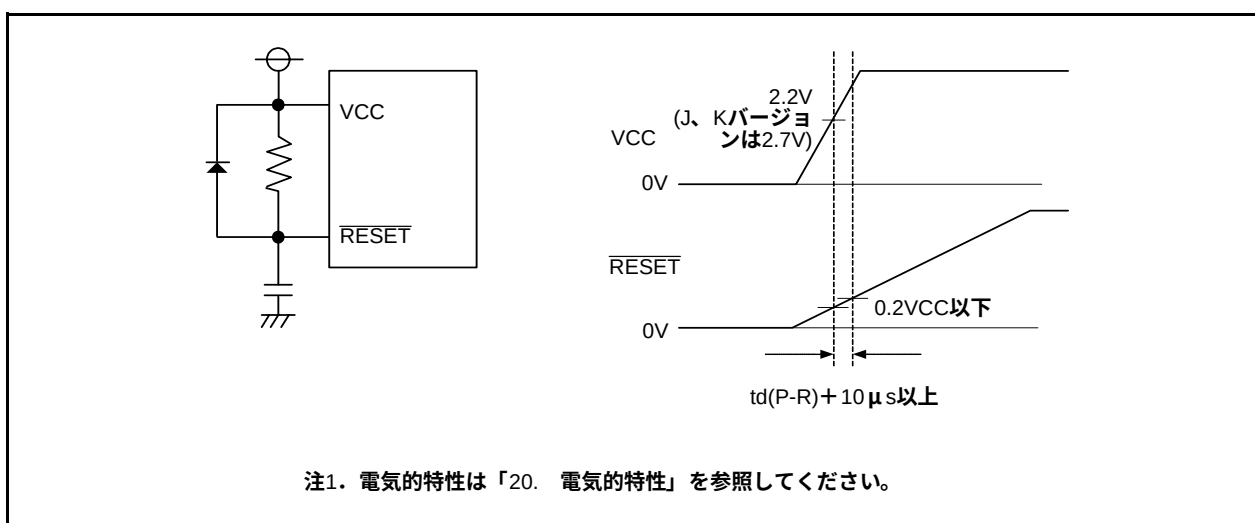
図5.6 ハードウェアリセット回路例と動作
