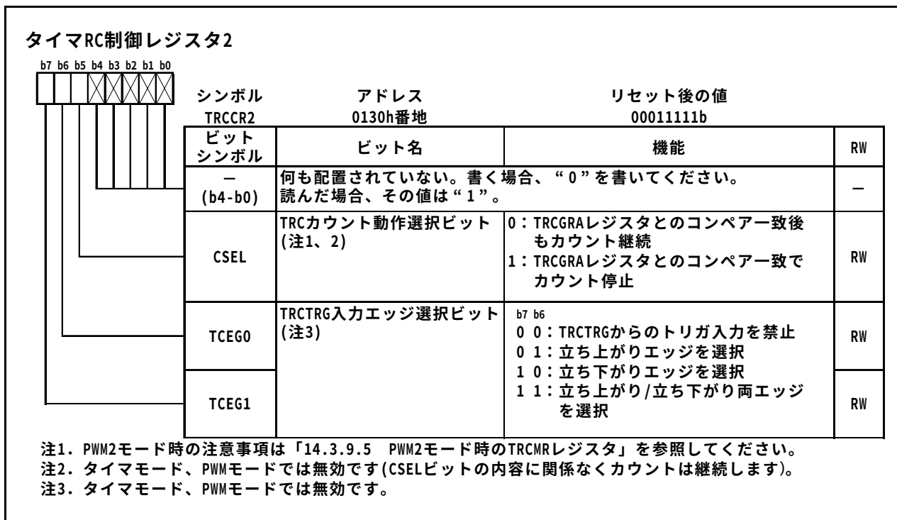
図14.33 TRCCR2レジスタ
