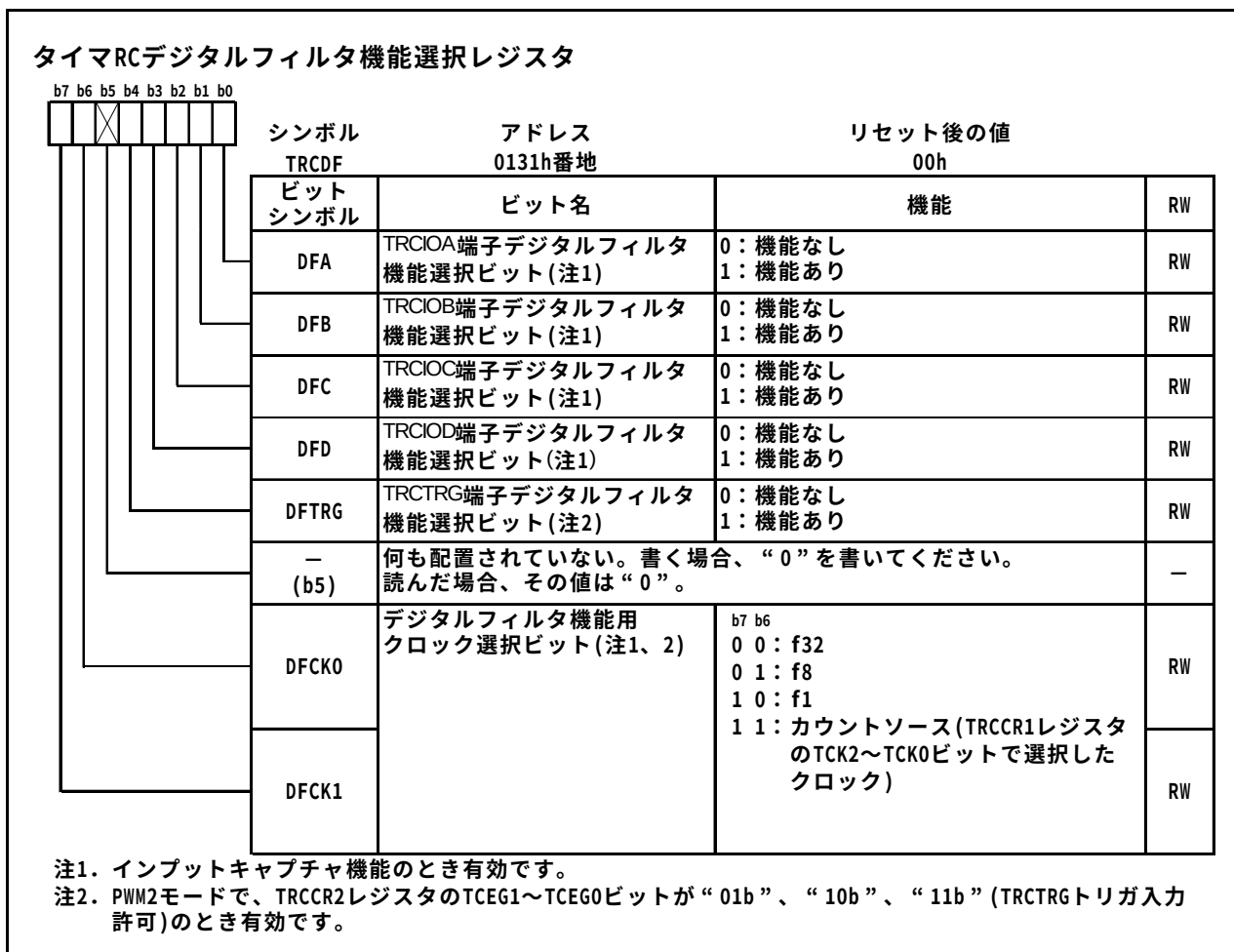
図14.34 TRCDFレジスタ
