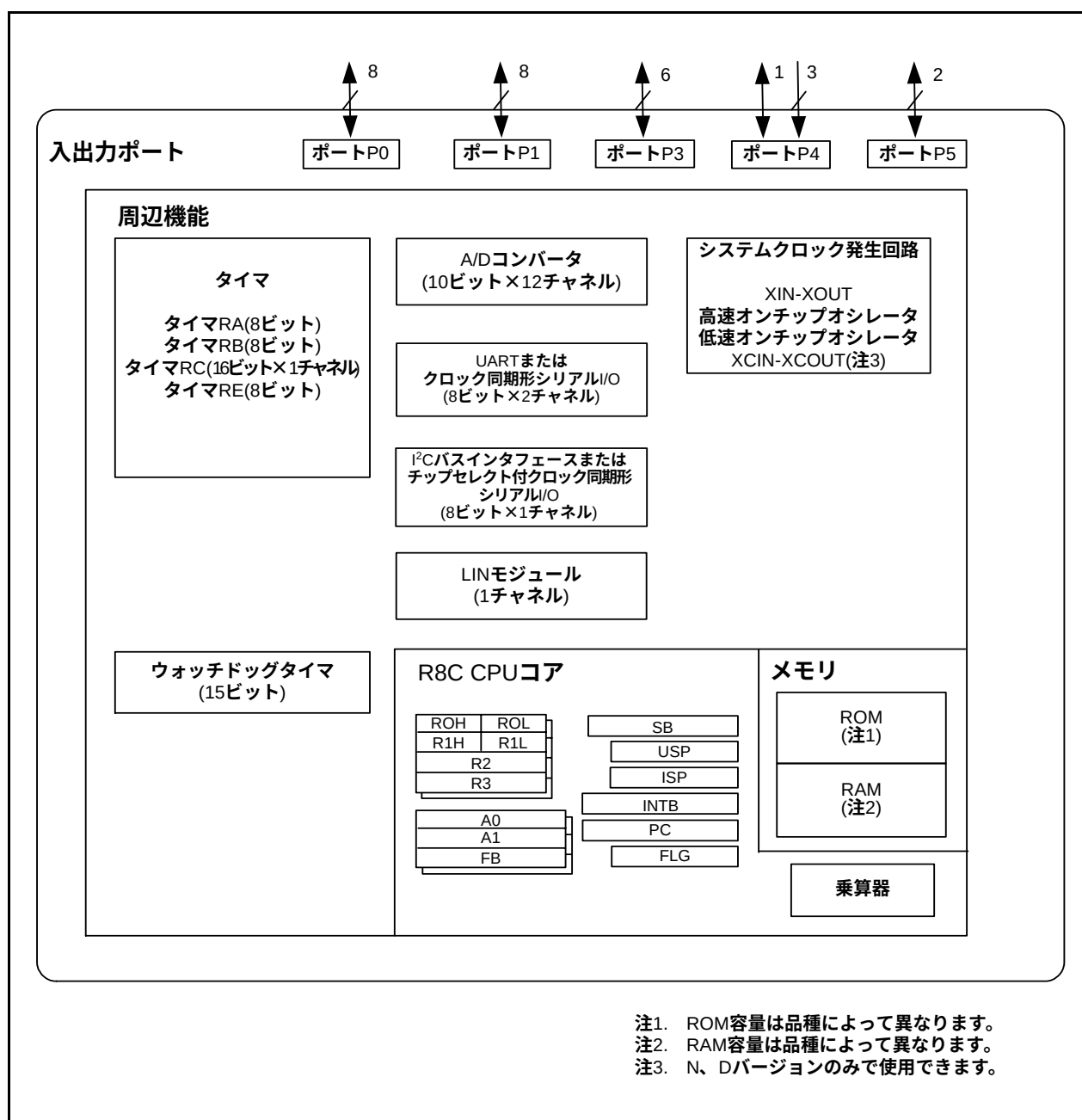
図1.1 ブロック図
