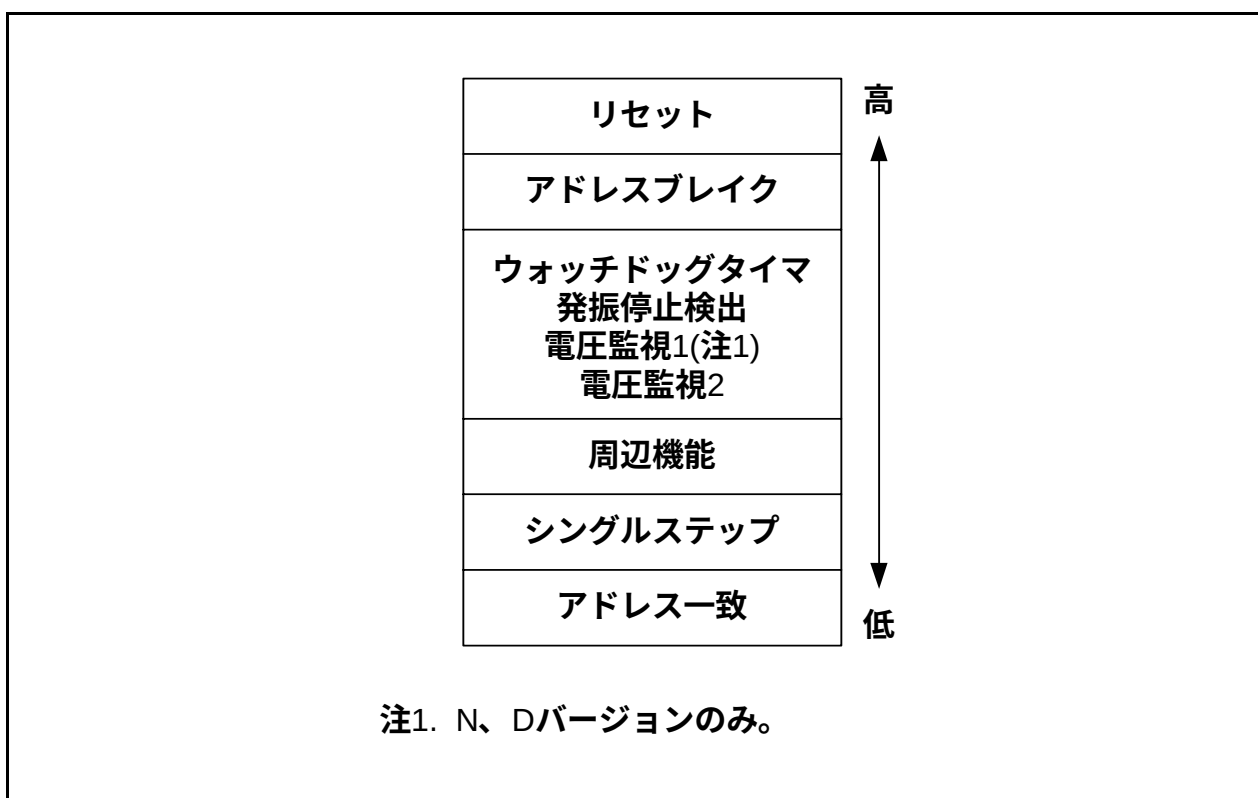
図12.10 ハードウェア割り込みの割り込み優先順位
