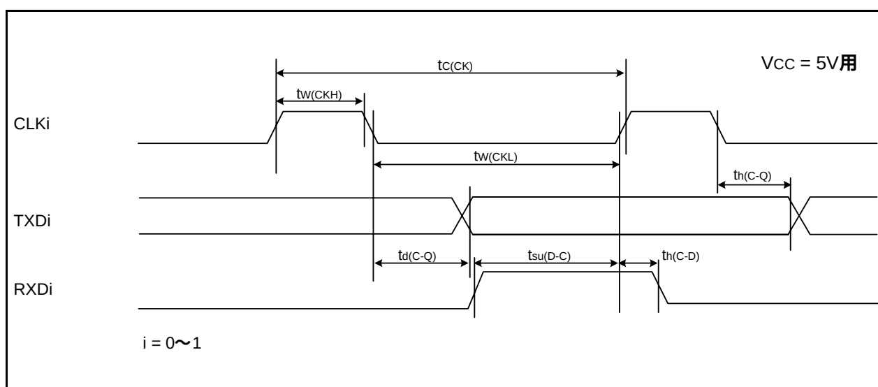
図 20.29 Vcc = 5V時のシリアルインタフェースのタイミング
