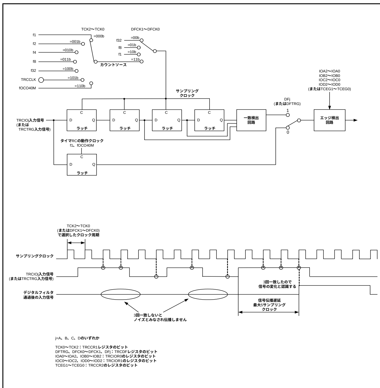
図14.40 デジタルフィルタのブロック図
