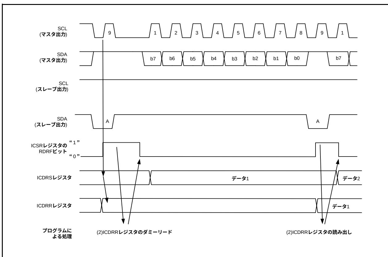
図 16.38 スレーブ受信モードの動作タイミング (I²C バスインタフェースモード) (1)
