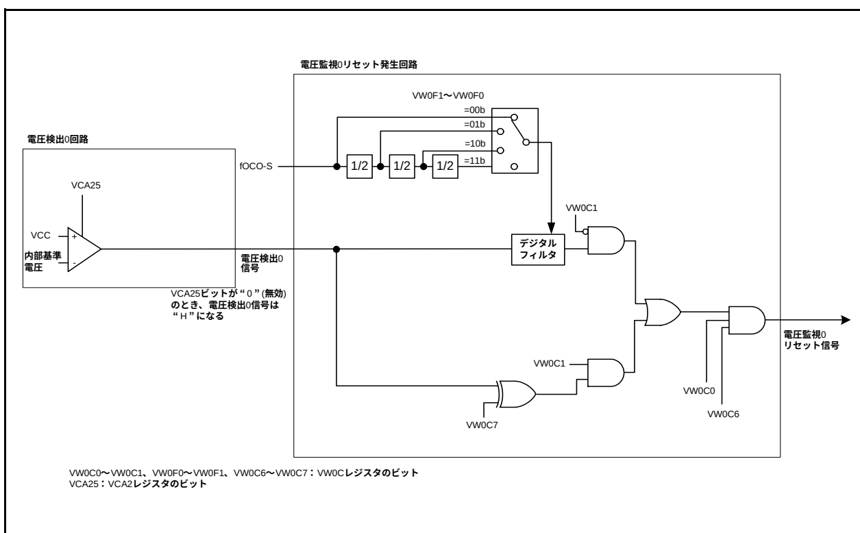
図6.3 電圧監視0リセット発生回路のブロック図(N、Dバージョンのみ)
