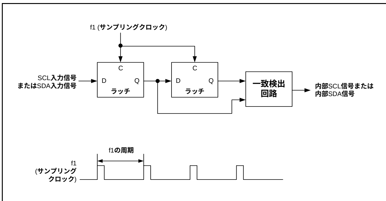
図16.43 ノイズ除去回路のブロック図
