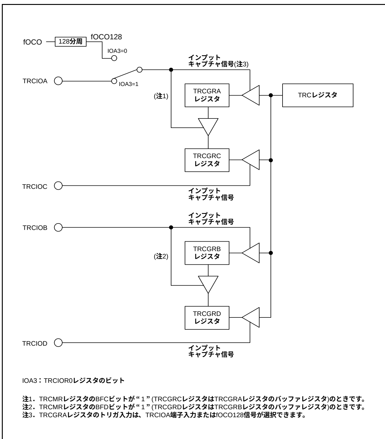
図14.42 インพุットキャプチャ機能のブロック図
