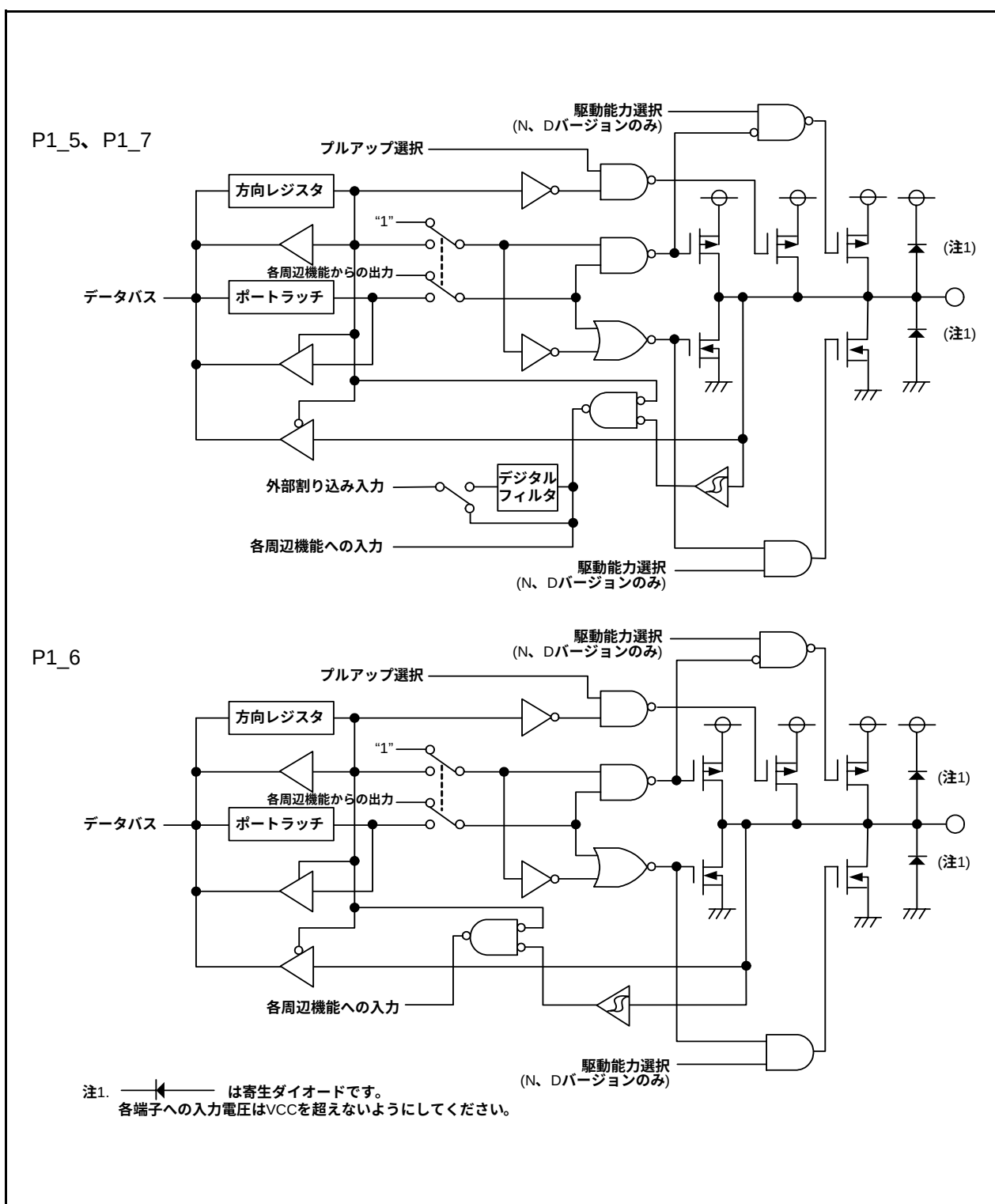
図7.2 プログラマブル入出力ポートの構成(2)
