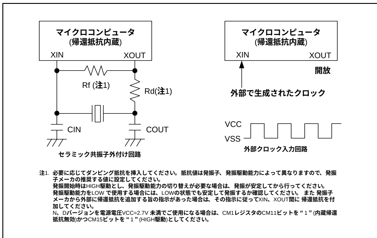
図10.11 XINクロックの接続回路例
