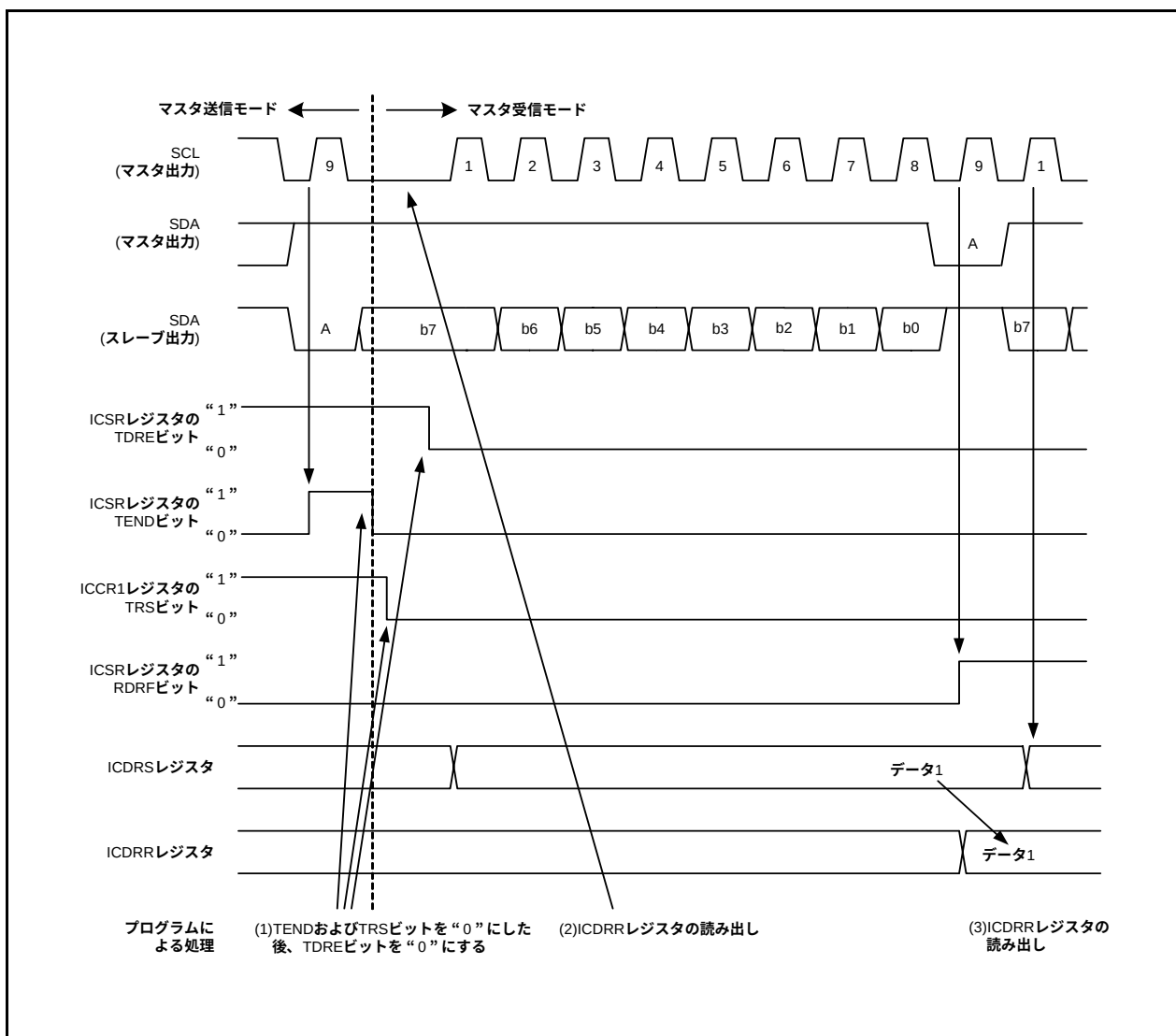
図16.34 マスタ受信モードの動作タイミング(I²Cバスインタフェースモード)(1)
