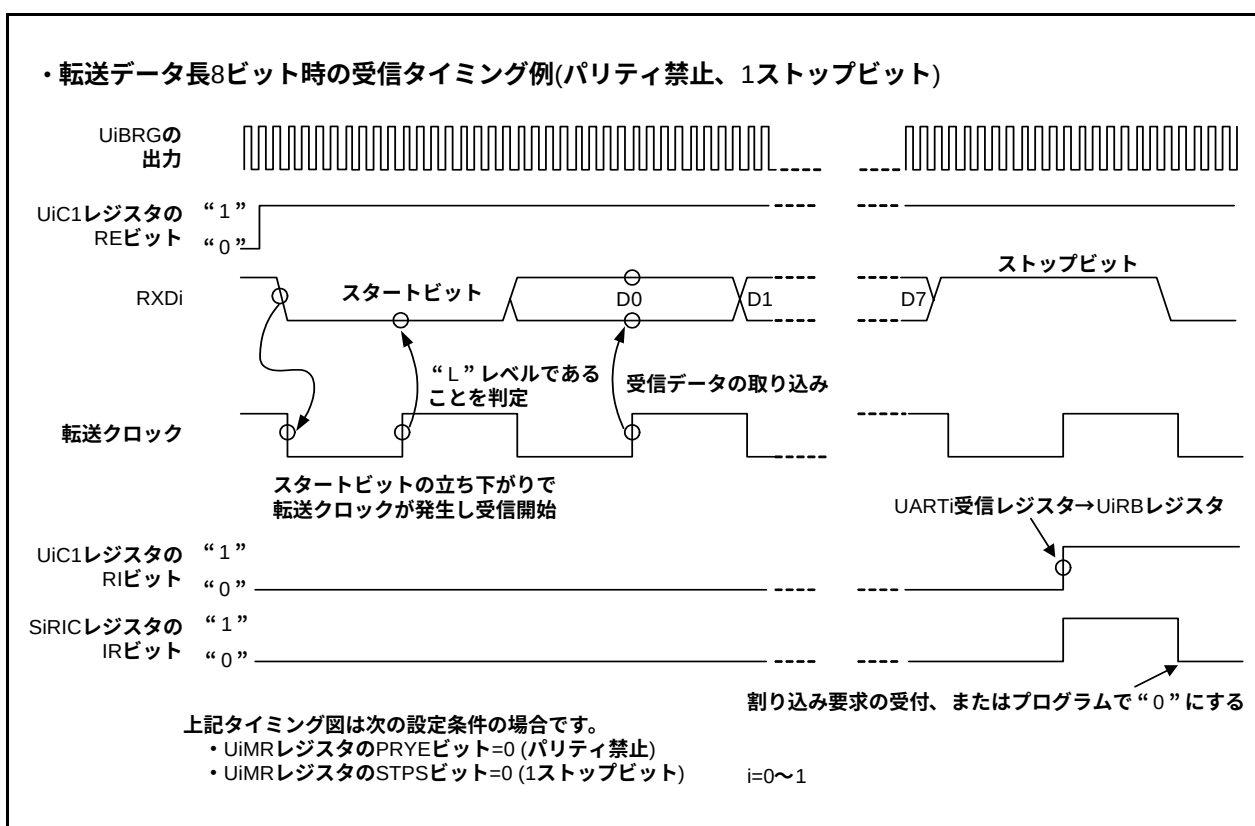
図 15.12 UART モード時の受信タイミング例
