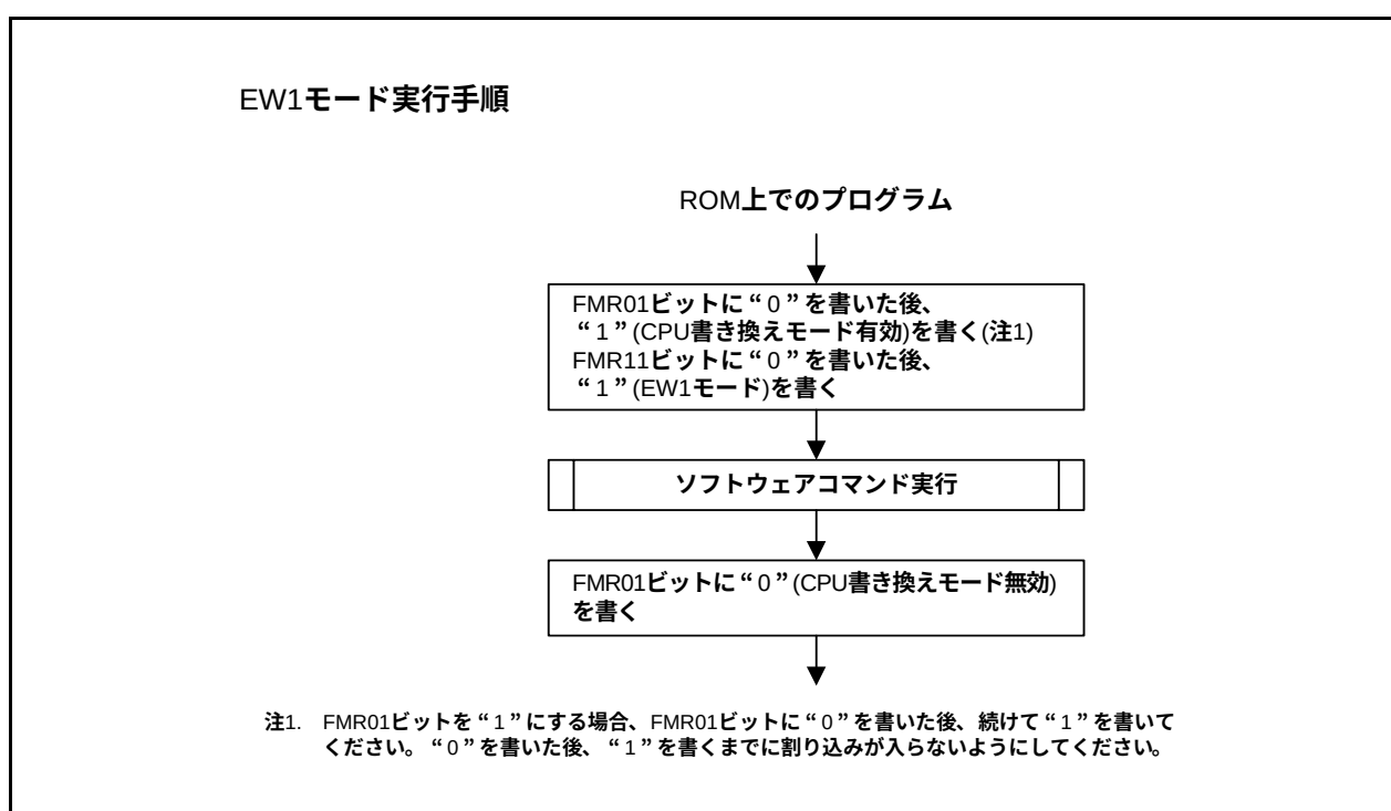
図19.10 EW1モードの設定と解除方法
