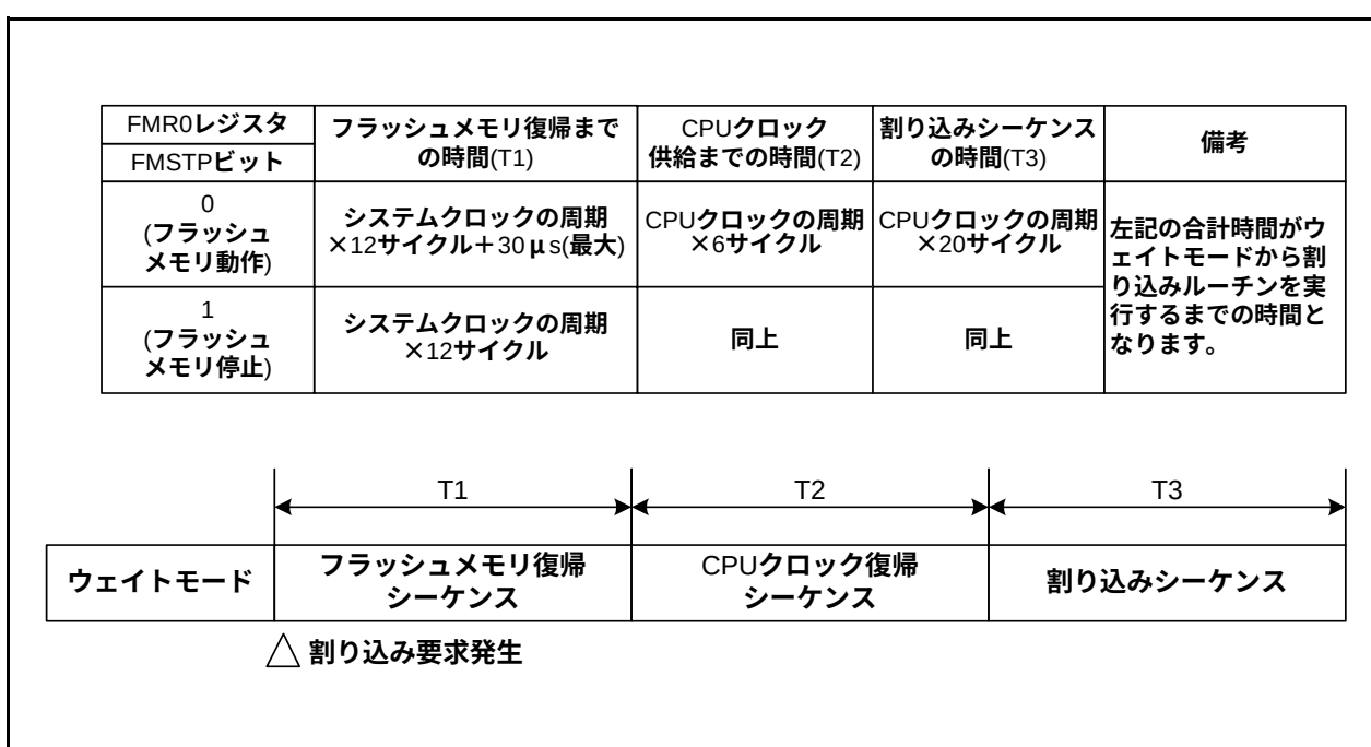
図10.13 ウェイトモードから割り込みルーチンを実行するまでの時間
