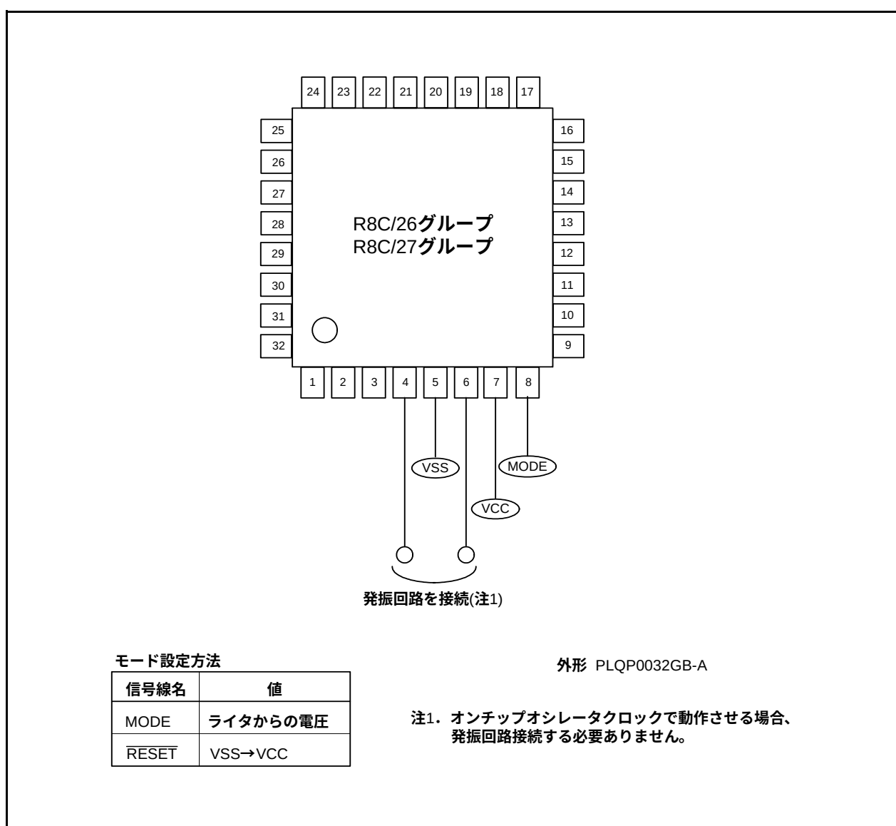
図19.17 標準シリアル入出力モード3時の端子結線図
