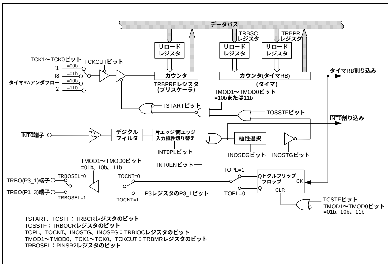
図14.12 タイマRBのブロック図
