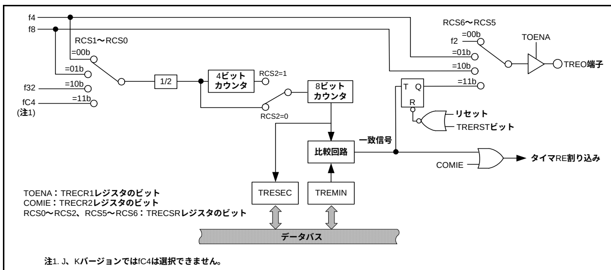
図 14.71 アウトプットコンペアモードのブロック図
