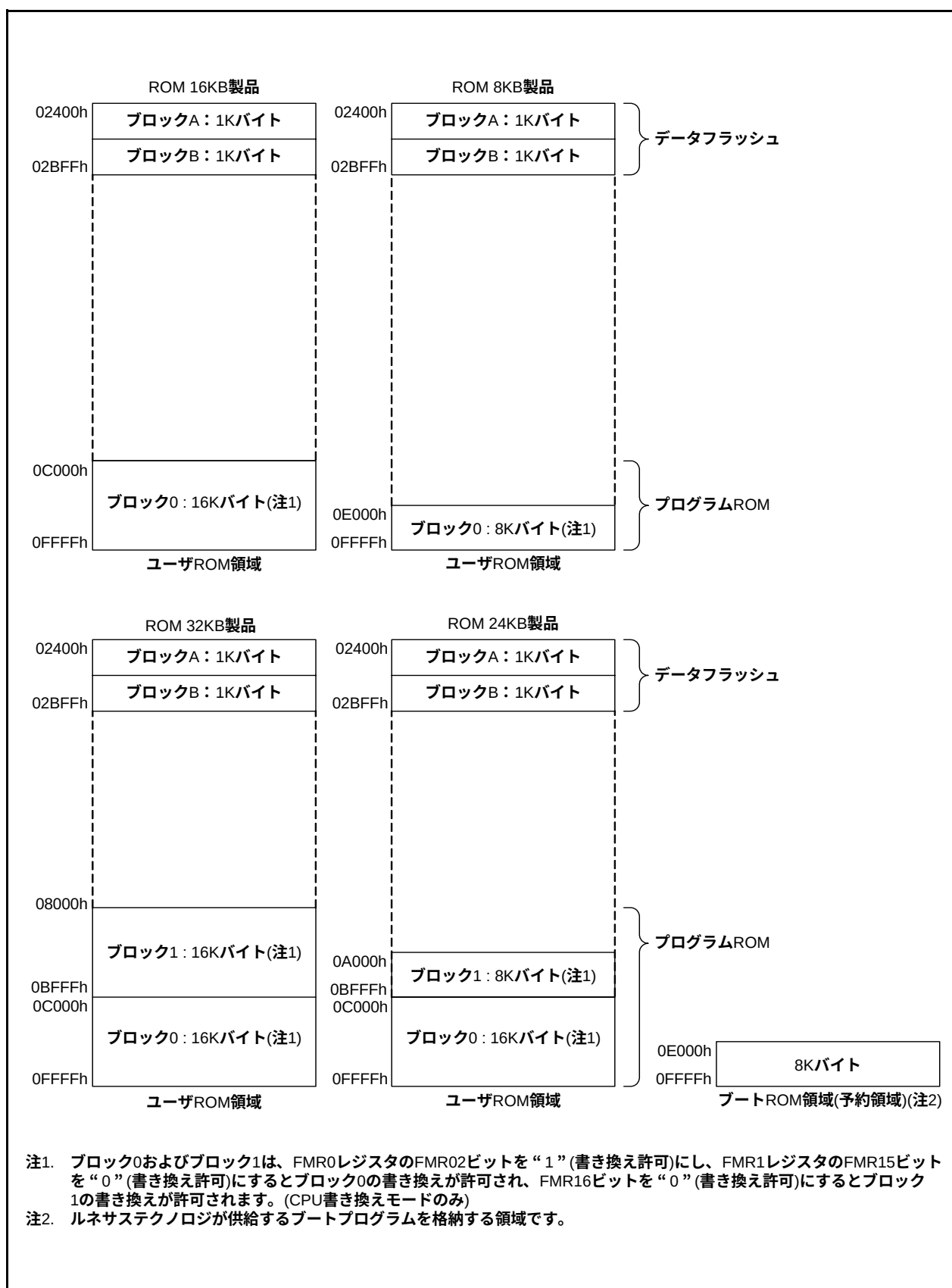
図 19.2 R8C/27グループのフラッシュメモリのブロック図
