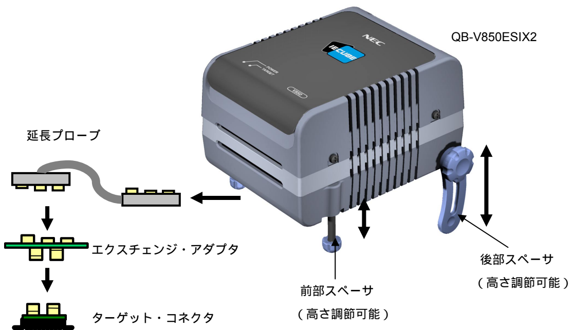
図2 - 8 延長プローブを使用する場合の接続
