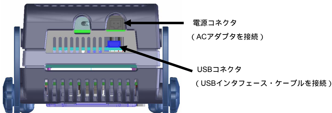
図2 - 9 コネクタ位置
