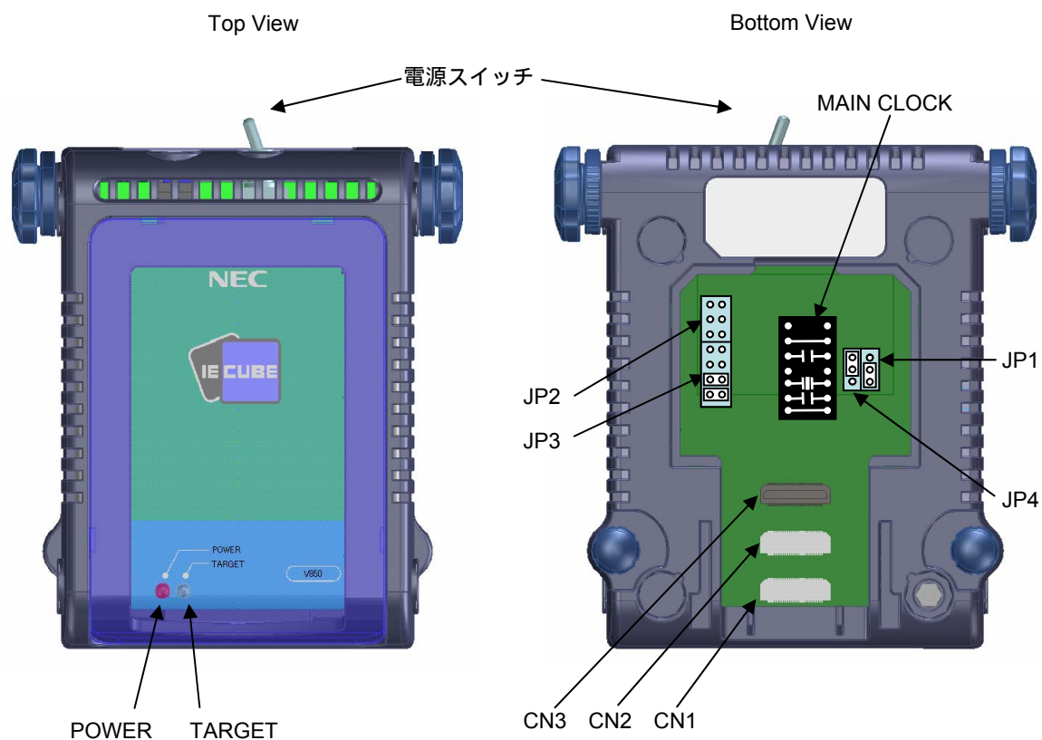
図2 - 1 QB-V850ESIX2の各部の名称
