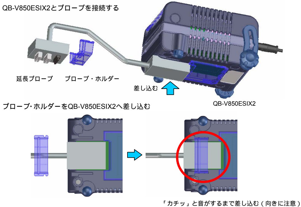
図2 - 5 プローブ・ホルダーの使用方法
