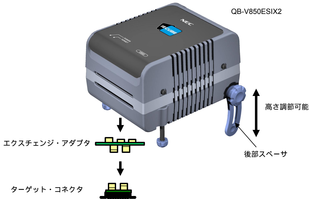
図2 - 4 延長プローブを使用しない場合の接続
