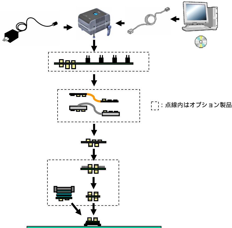
図1-1 システム構成（Sタイプ）
