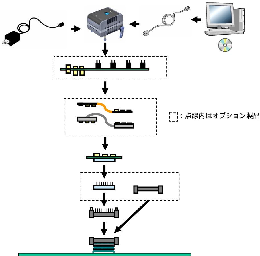
図1-2 システム構成 (Tタイプ)
