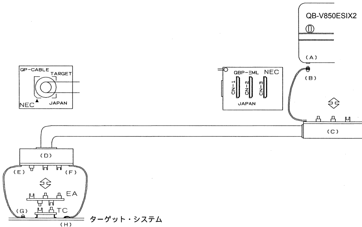
図2-6 GND線
