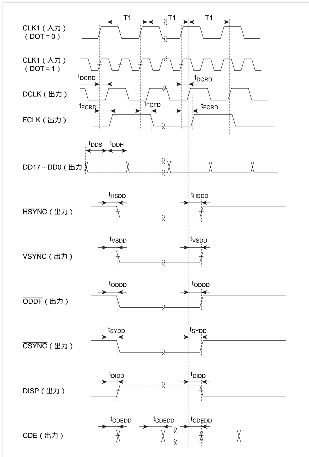
図 7.13 マスタモード表示タイミング
