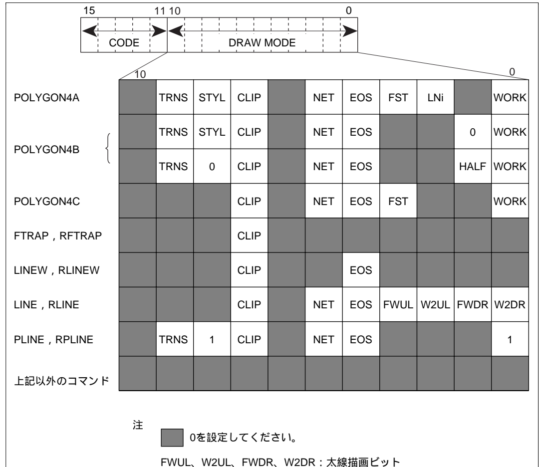
図 4.13 レンダリング属性のビット配置
