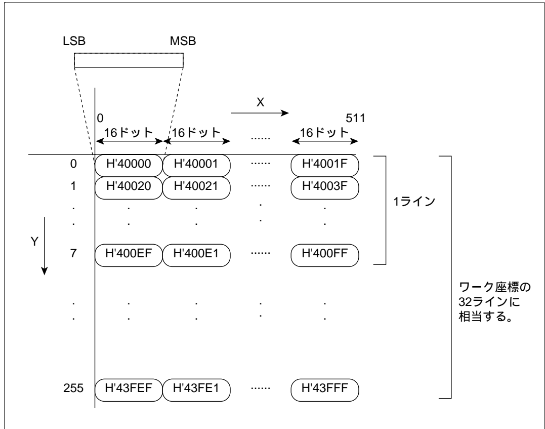
図 4.8 ワーク座標の座標対アドレスの関係
