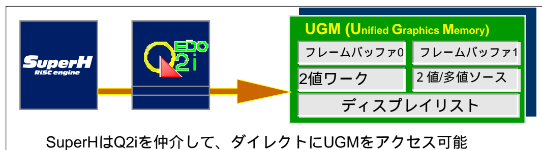
図 1.4 システムバスインタフェースの一元化 ( SuperH は Q2i を仲介して、ダイレクトに UGM をアクセス可能 )
