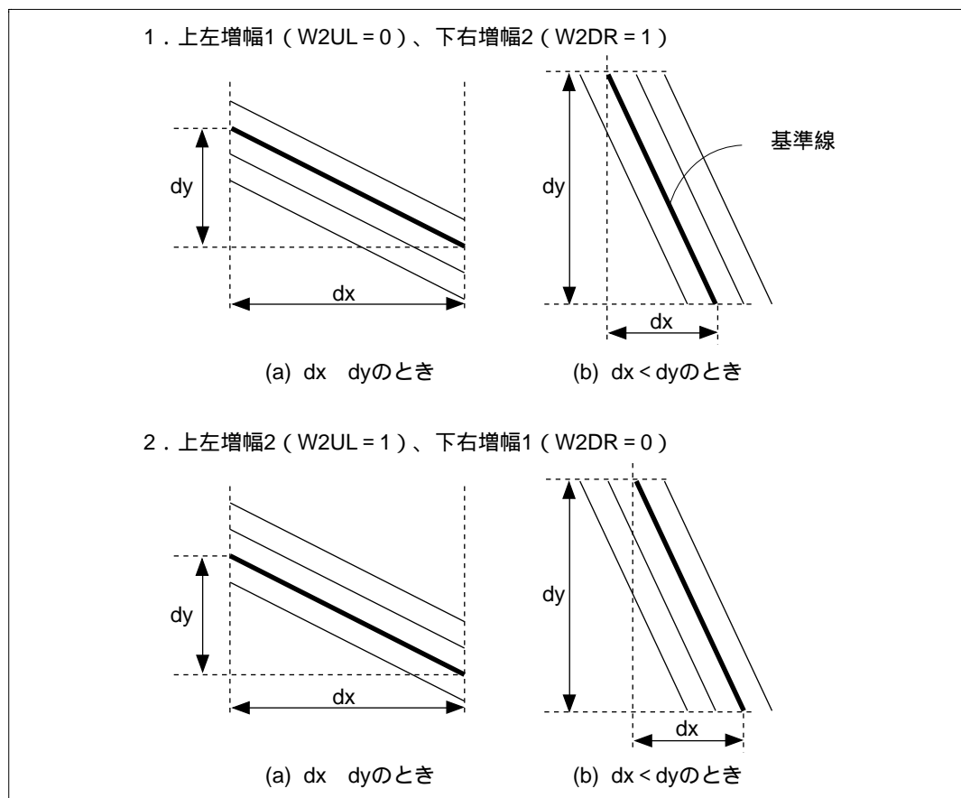
図 4.17 太線描画の例 (線幅 4 の描画例) ただし、FWUL = 1 かつ FWDR = 1
