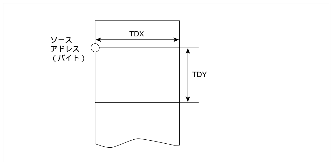
図 4.4 LNi = 1 指定時の多値ソース座標 (リニアアドレス)
