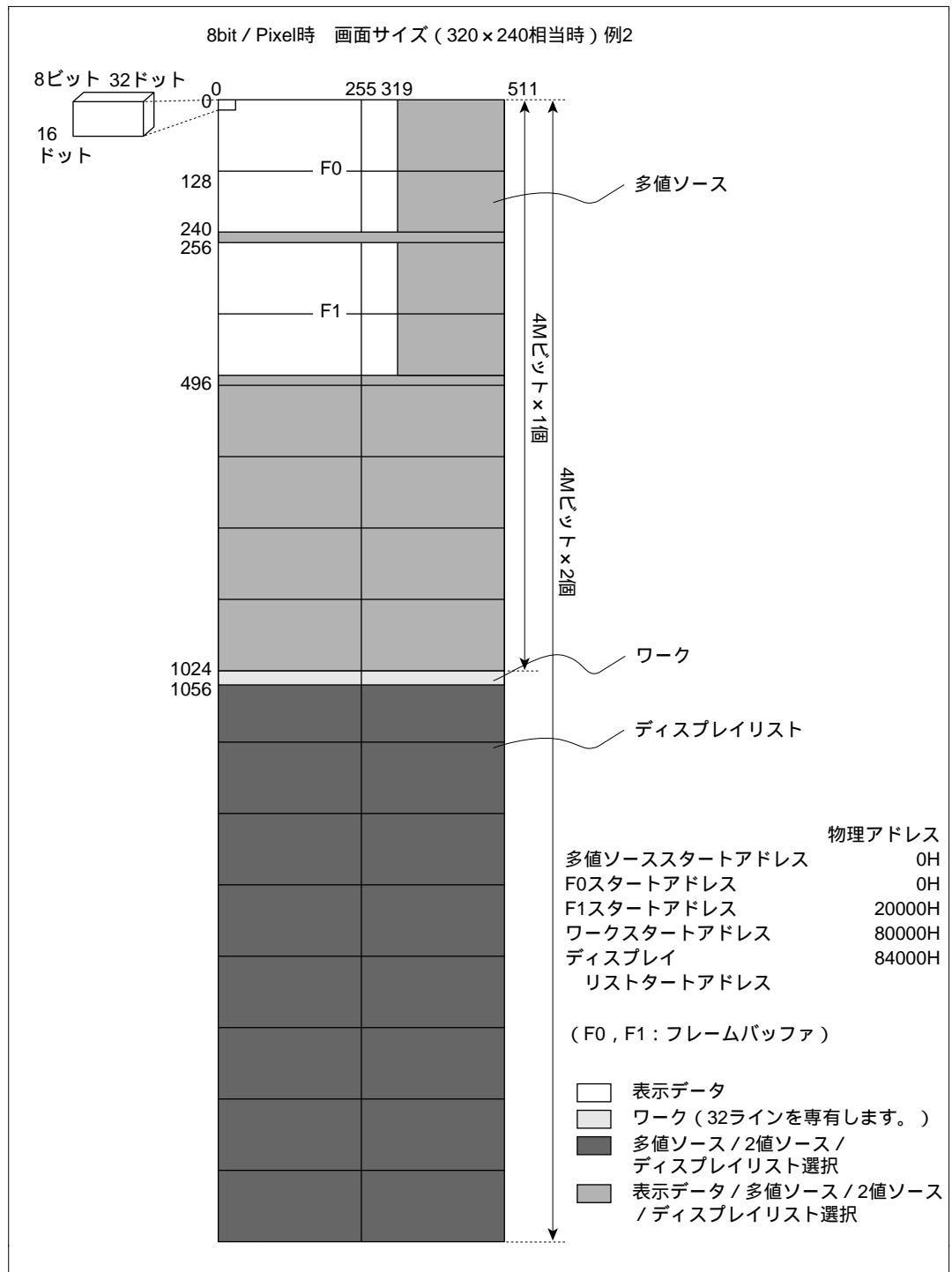
図 3.5 メモリマップ例2 [8ビット/画素時 画面サイズ (320 × 240 相当時) ]
