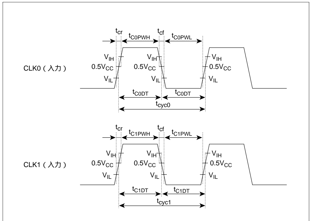
図 7.3 入力クロック (MODE2 ~ MODE0 端子 = "011" のとき)
