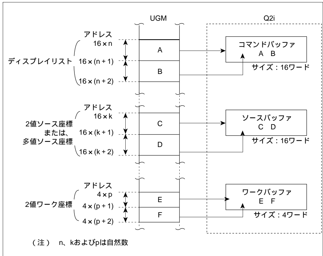
図 6.3 Q2i 内のバッファの更新
