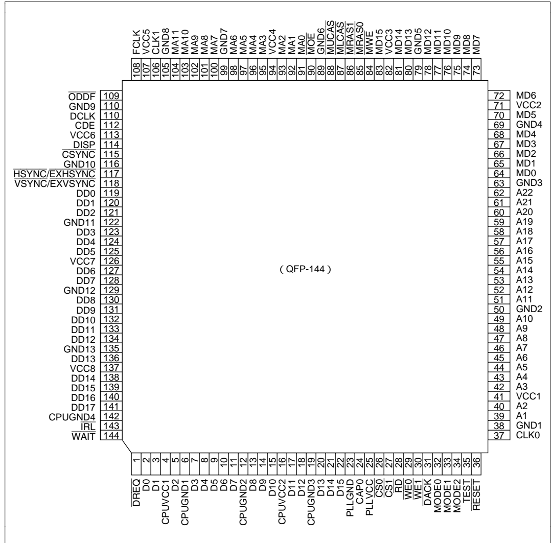
図 2.2 ピン配置図
