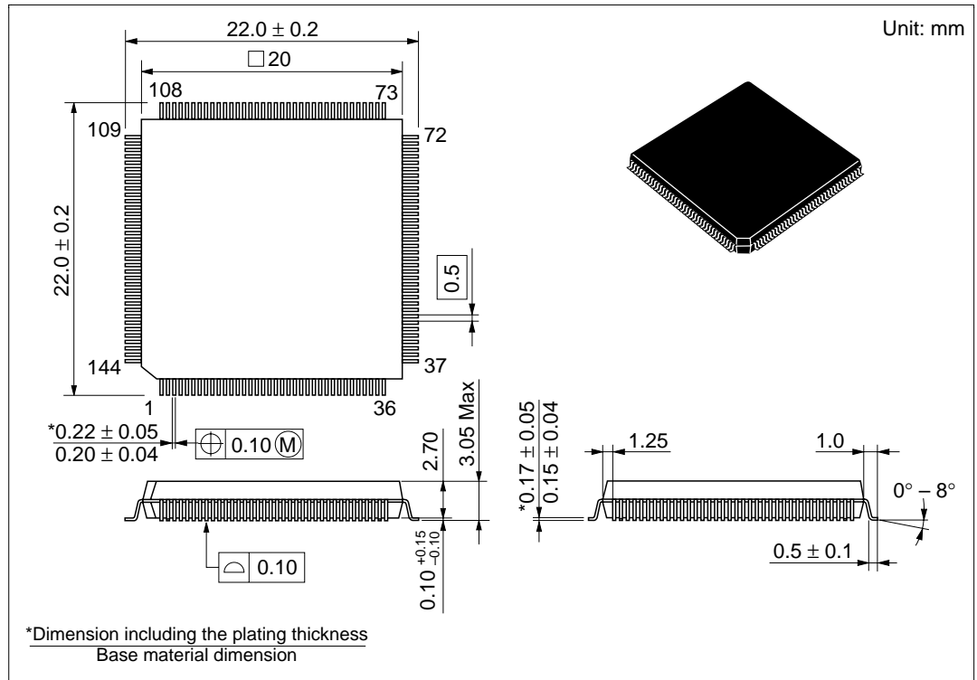
図 D.1 パッケージ外形寸法図 (FP-144)
