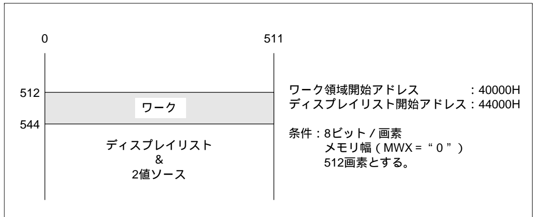
図 4.7 ワーク座標と物理アドレスの関係例
