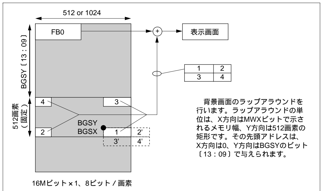
図 3.20 背景画面の球面スクロール (WRAP = " 1 " ) の例
