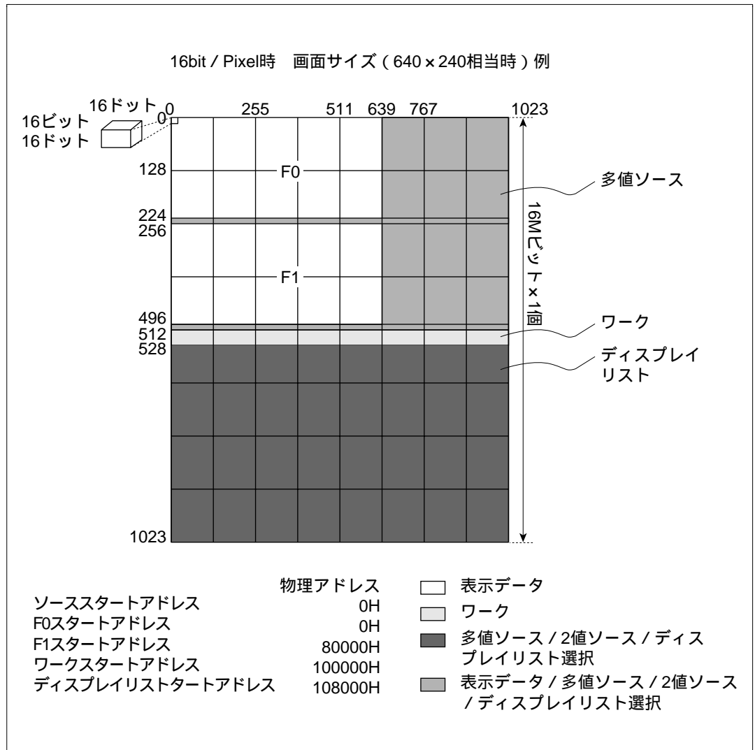
図 3.9 メモリマップ例 6 [ 16 ビット / 画素時 画面サイズ (640 × 240 相当時) ]
