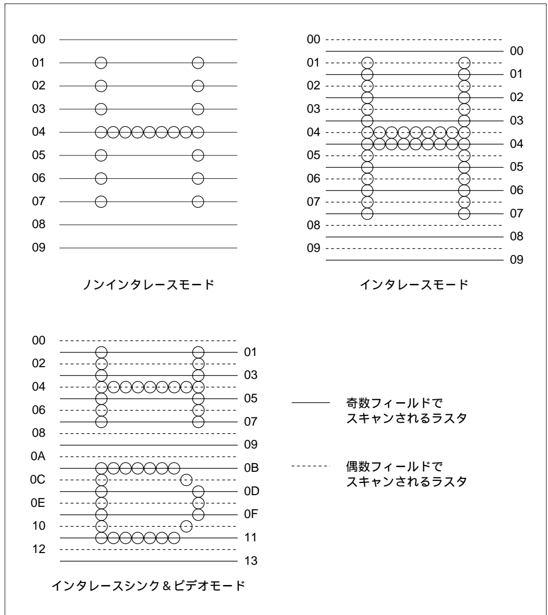
図 3.17 ラスタスキャン制御の表示例
