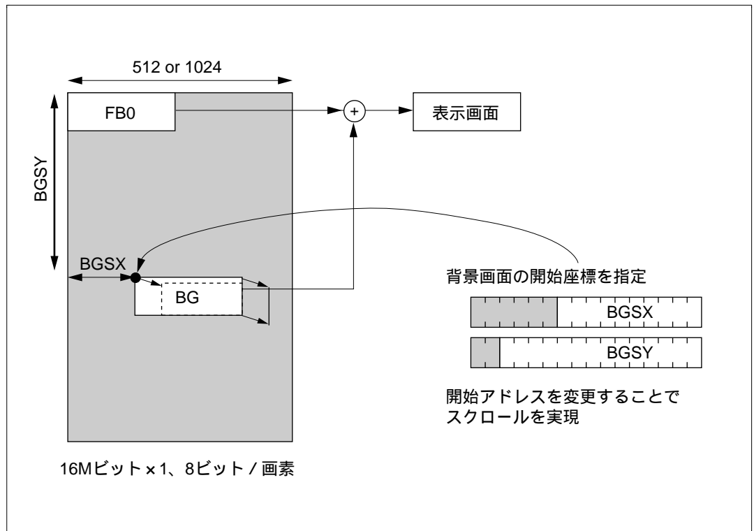
図 3.19 背景画面の単純スクロール (WRAP = " 0 " ) の例
