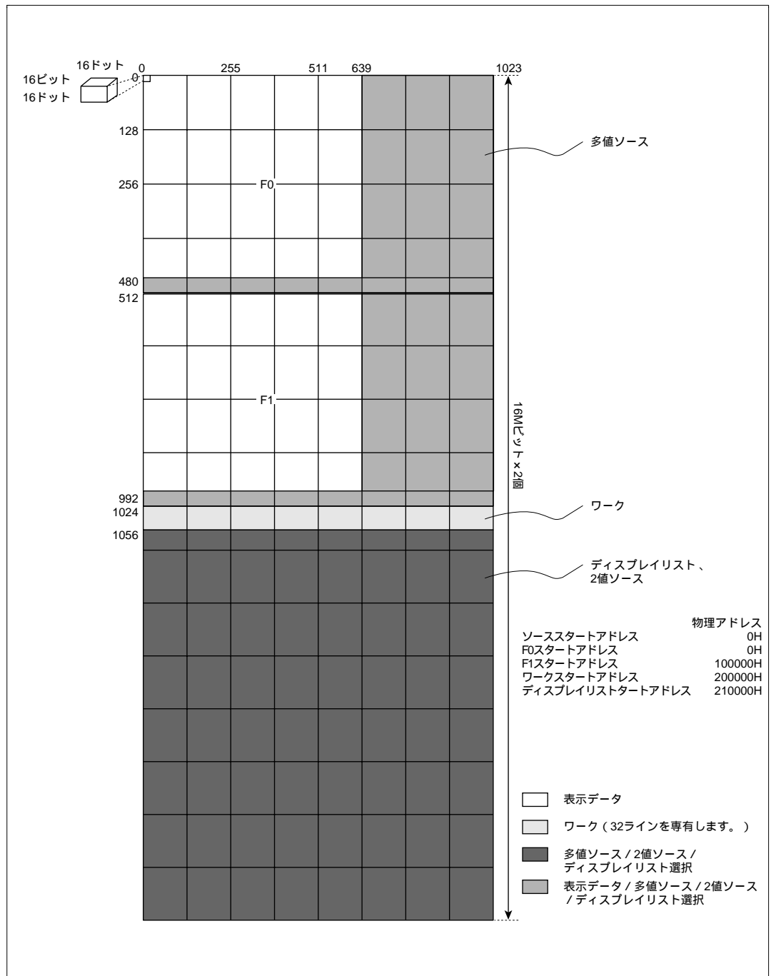
図 3.10 メモリマップ例7 [16ビット/画素時 画面サイズ(640×480相当時)]
