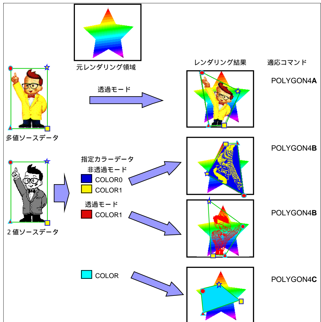
図 4.9 POLYGON4 系転送データの組み合わせ例
