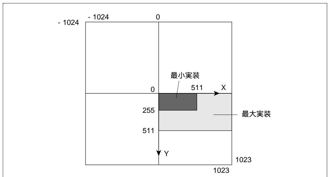
図 4.6 ワーク座標系
