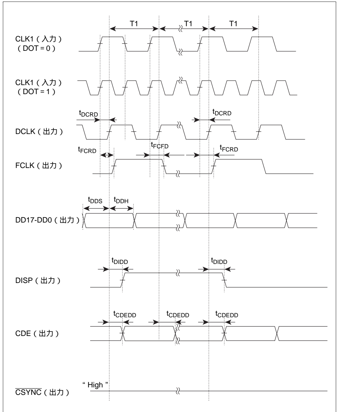
図 7.14 (1) TV 同期モード表示タイミング
