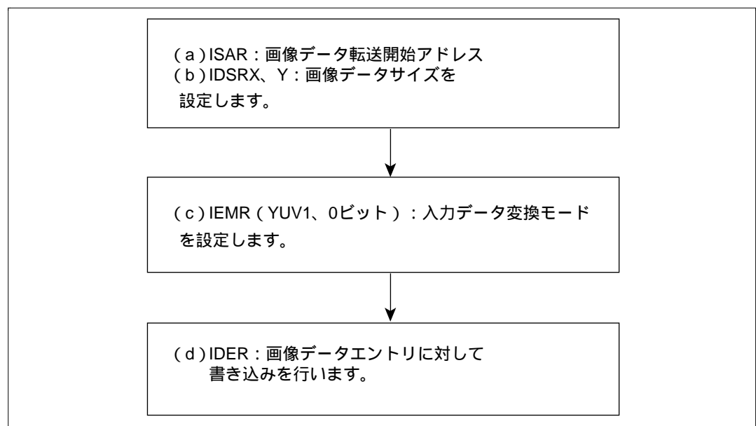
図 3.15 \Delta YUV、YUV RGB 変換時のレジスタ設定手順
