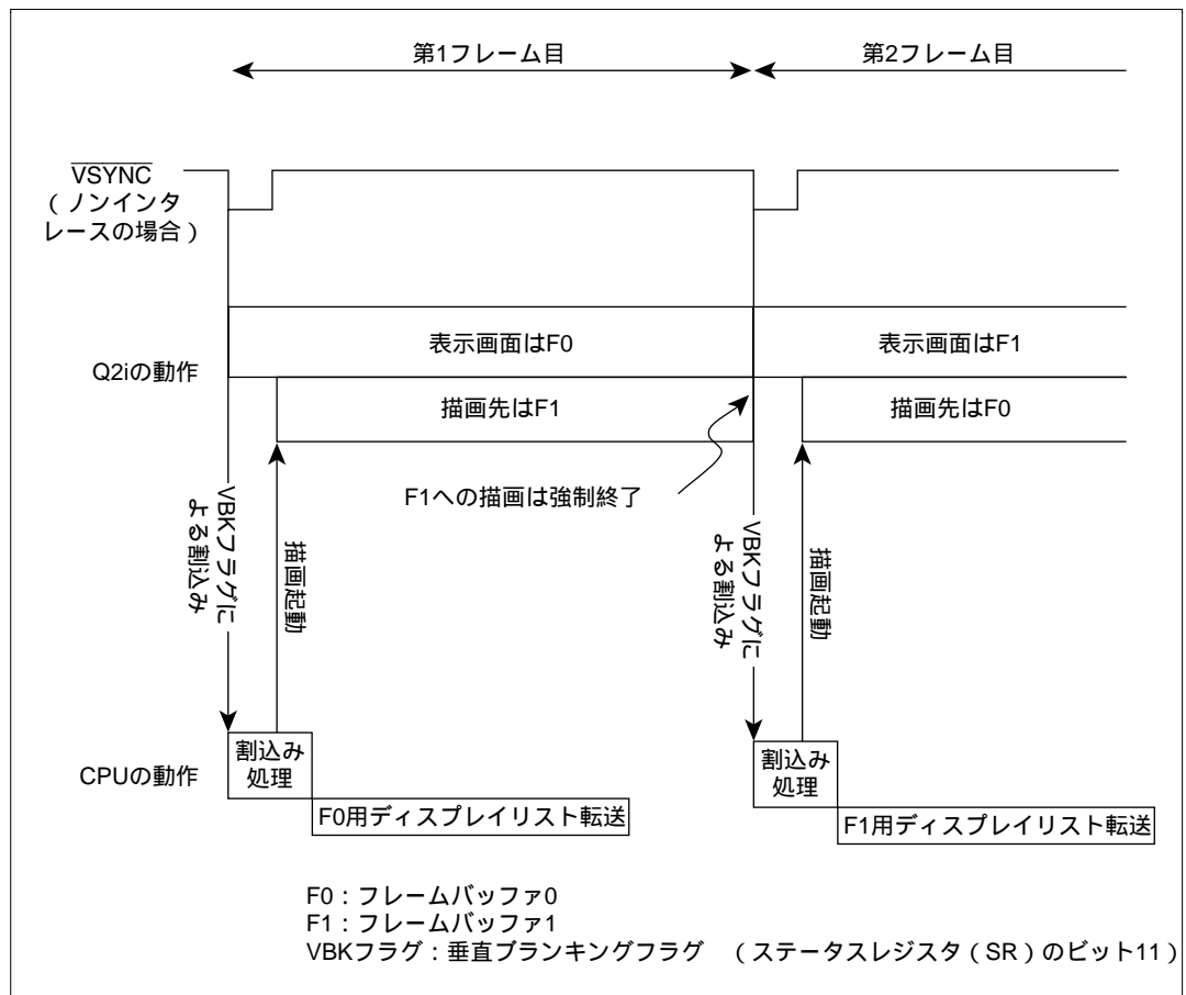
図 3.11 オートディスプレイチェンジモードの動作
