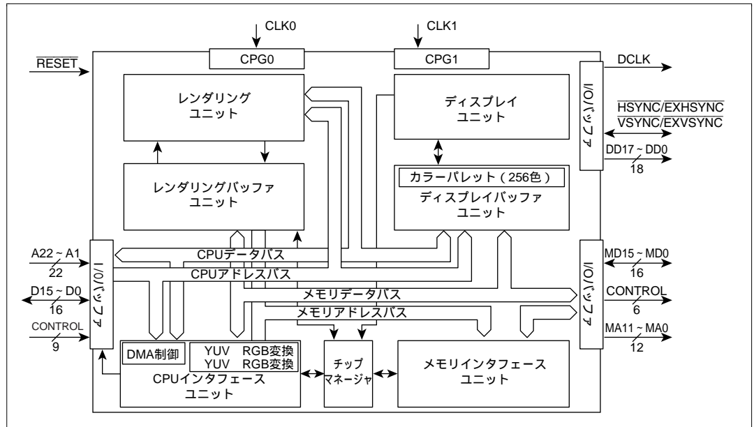
図 1.2 内部ブロック図
