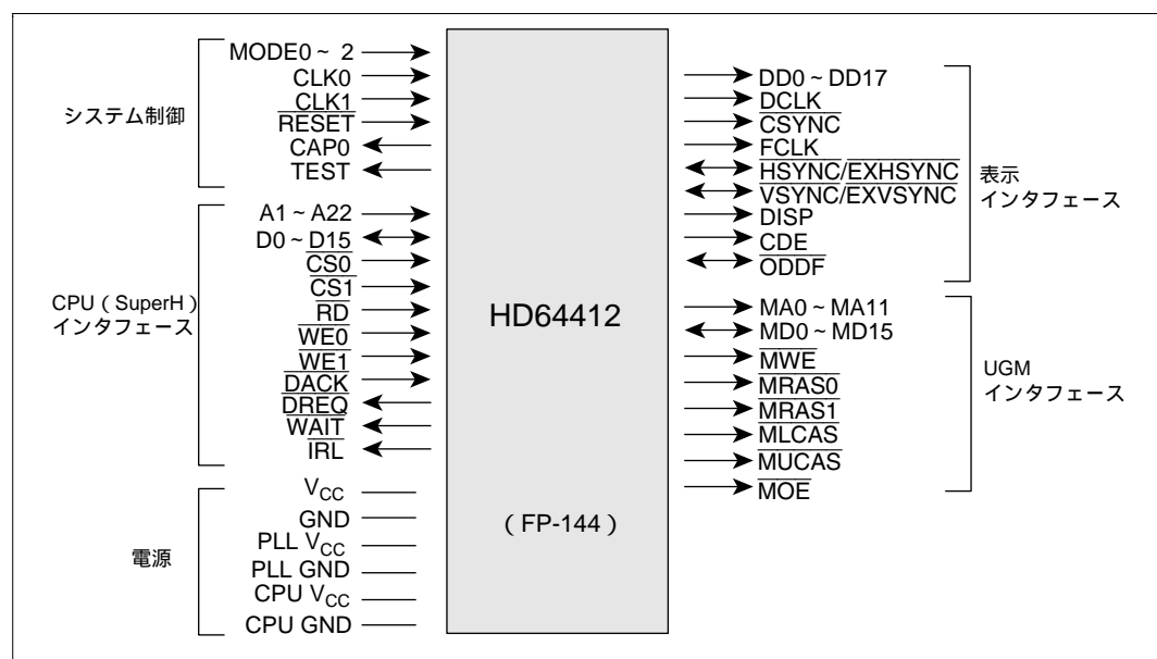
図 2.1 端子概要
