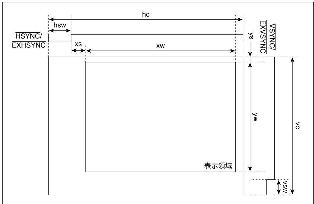
図 3.16 表示タイミング
