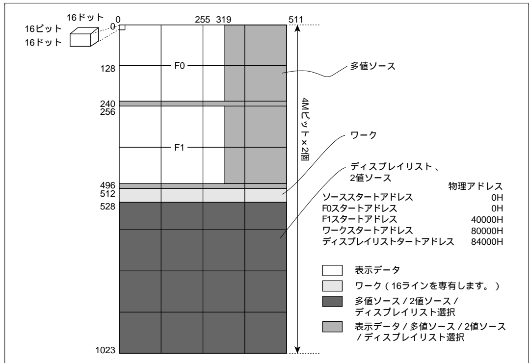
図 3.8 メモリマップ例 5 [ 16 ビット / 画素時 画面サイズ ( 320 × 240 相当時 ) ]
