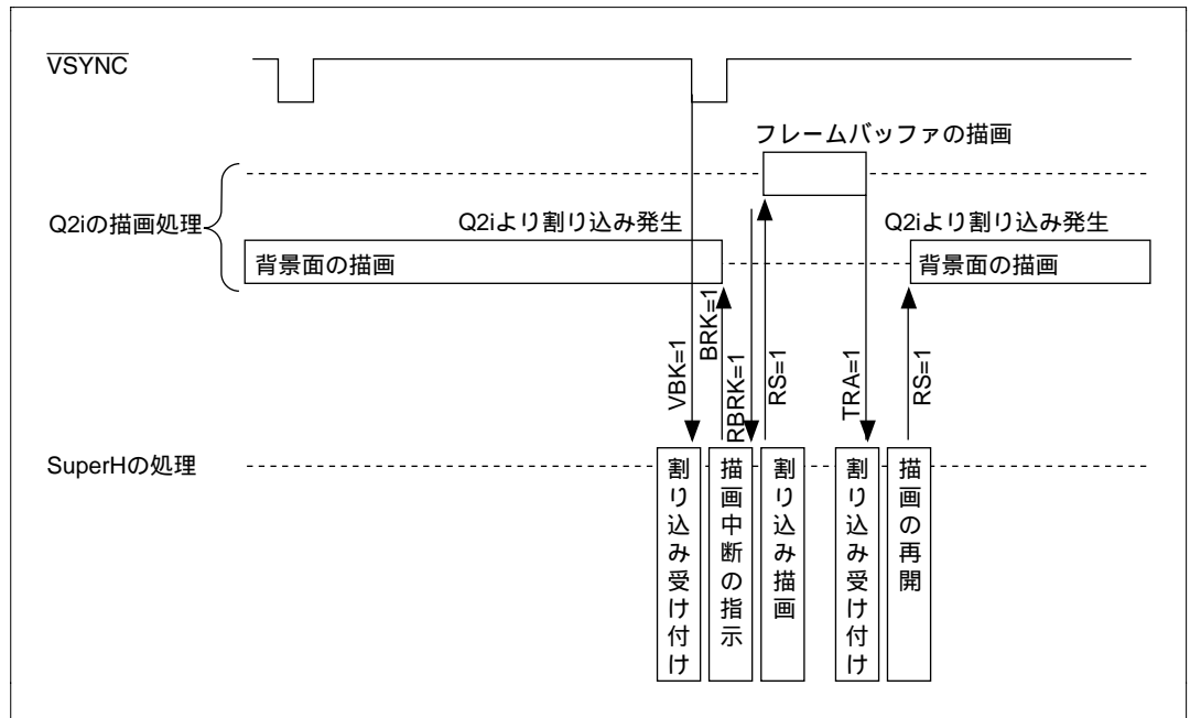
図 1.13 背景面に対する描画の中断・再開タイミング例
