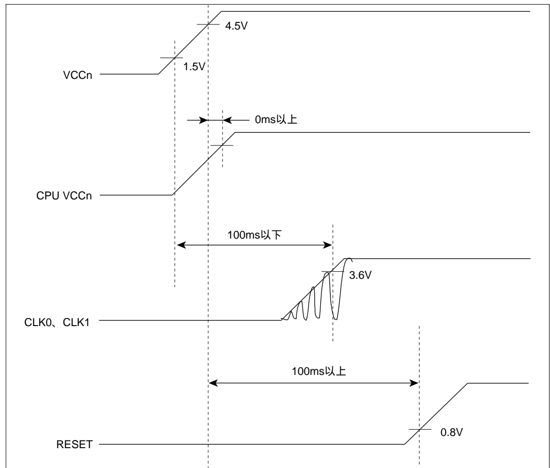
図 6.2 CLK0、CLK1、RESET 信号タイミング
