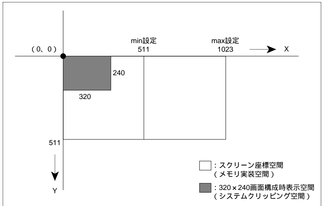
図 1.7 スクリーン座標
