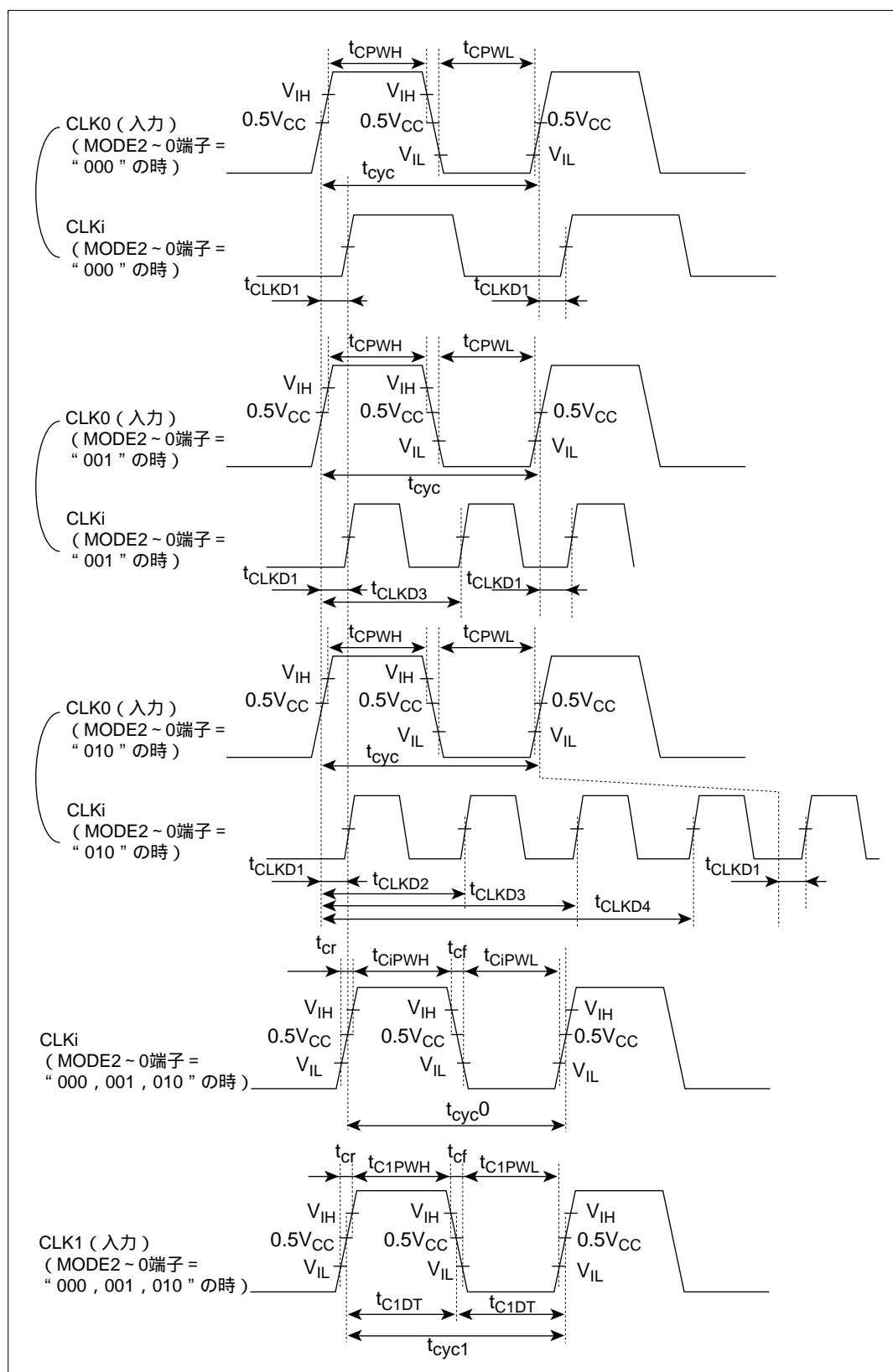
図 7.4 入力クロック (MODE2 ~ MODE0 端子 = "000、001、010" のとき)
