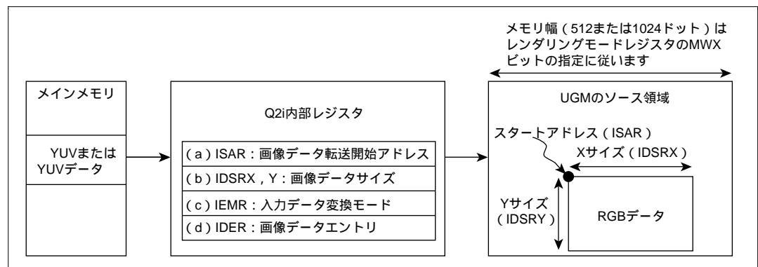
図 3.14 \Delta YUV、YUV RGB 変換機能の仕様
