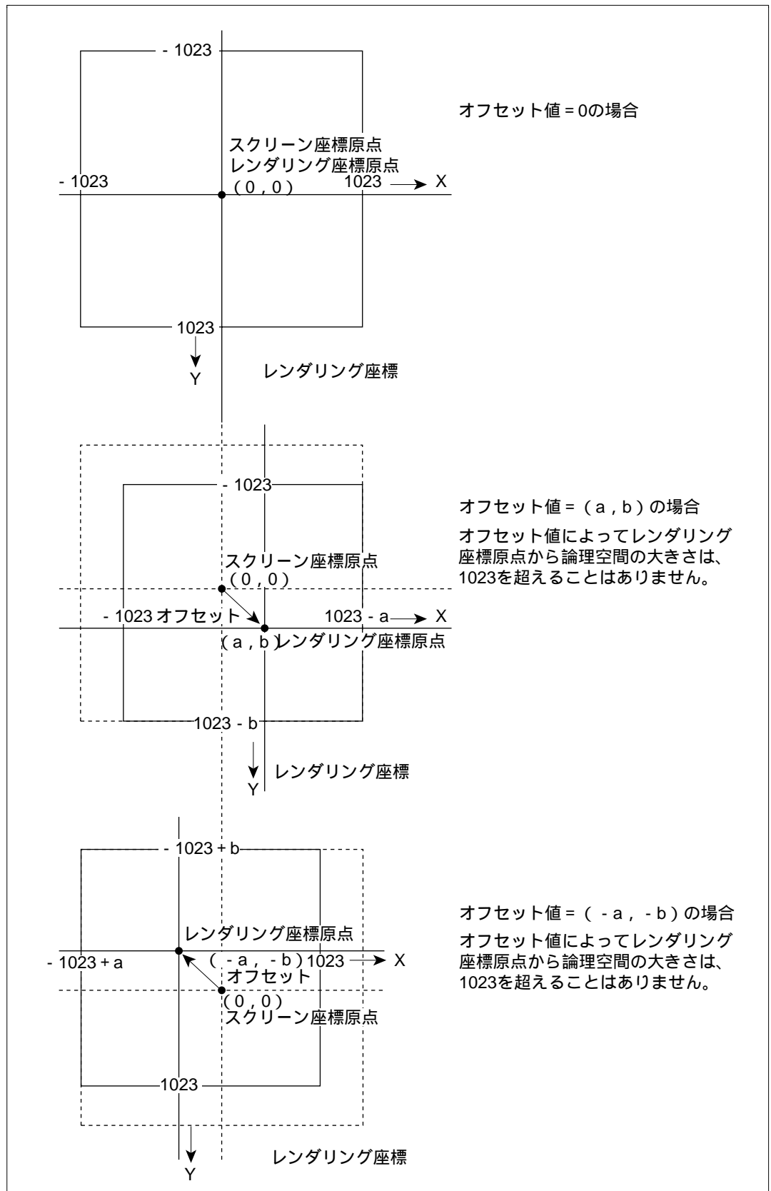
図 1.8 レンダリング座標
