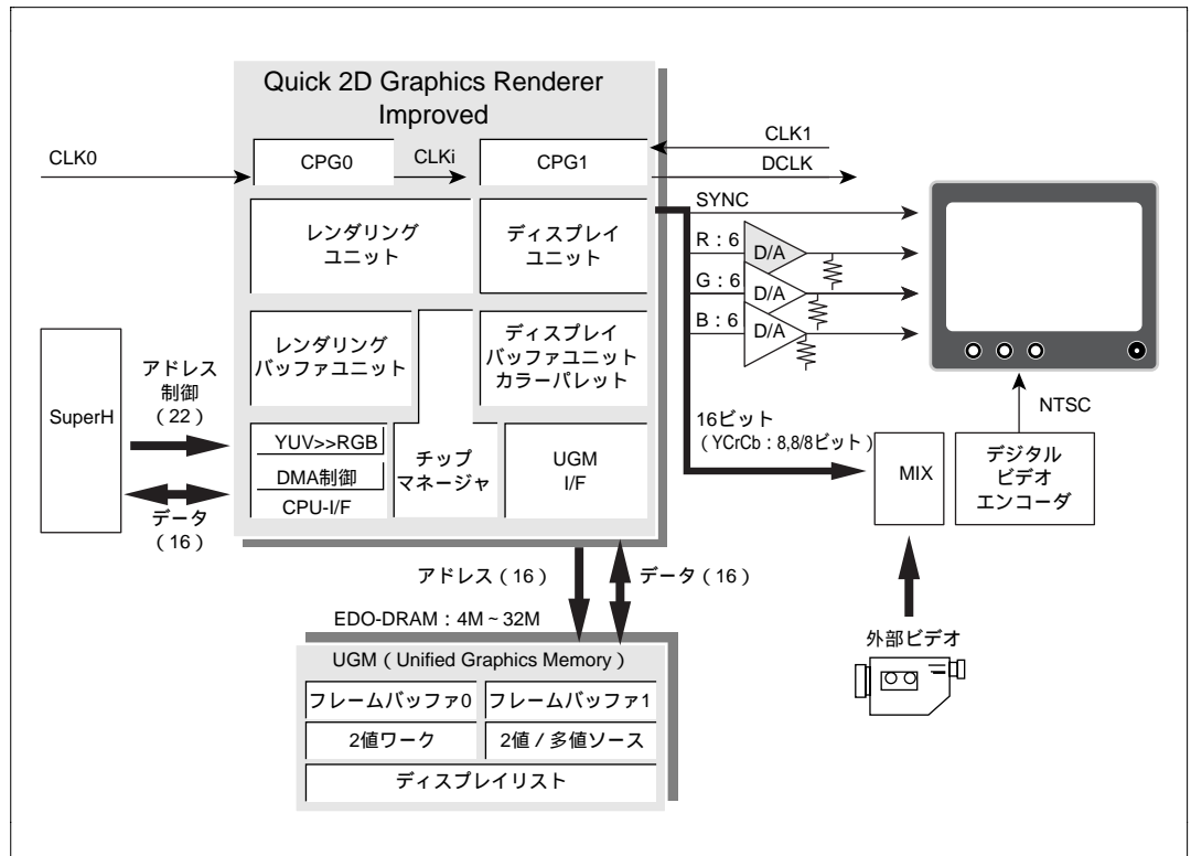
図 1.1 システム概要図
