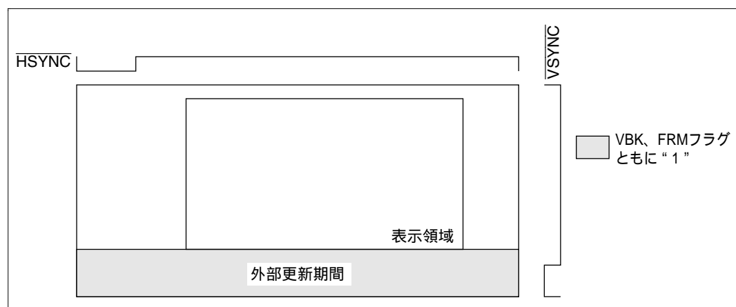
図5.1(a) 外部更新期間(ノンインタレース時)
