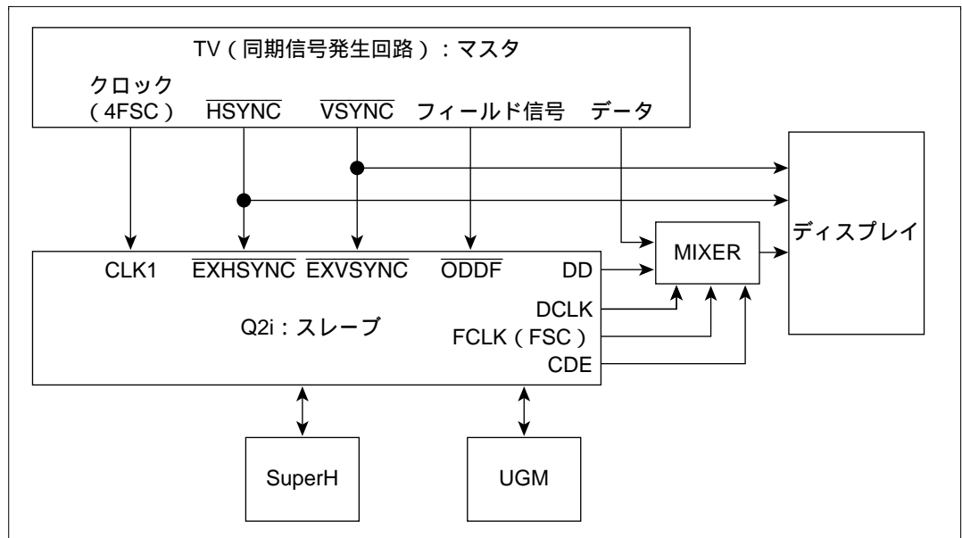
図 3.18 TV 同期モード時の信号の流れ
