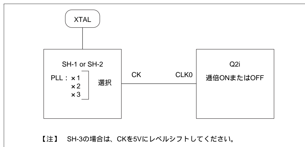
図 6.1 同期動作の接続例
