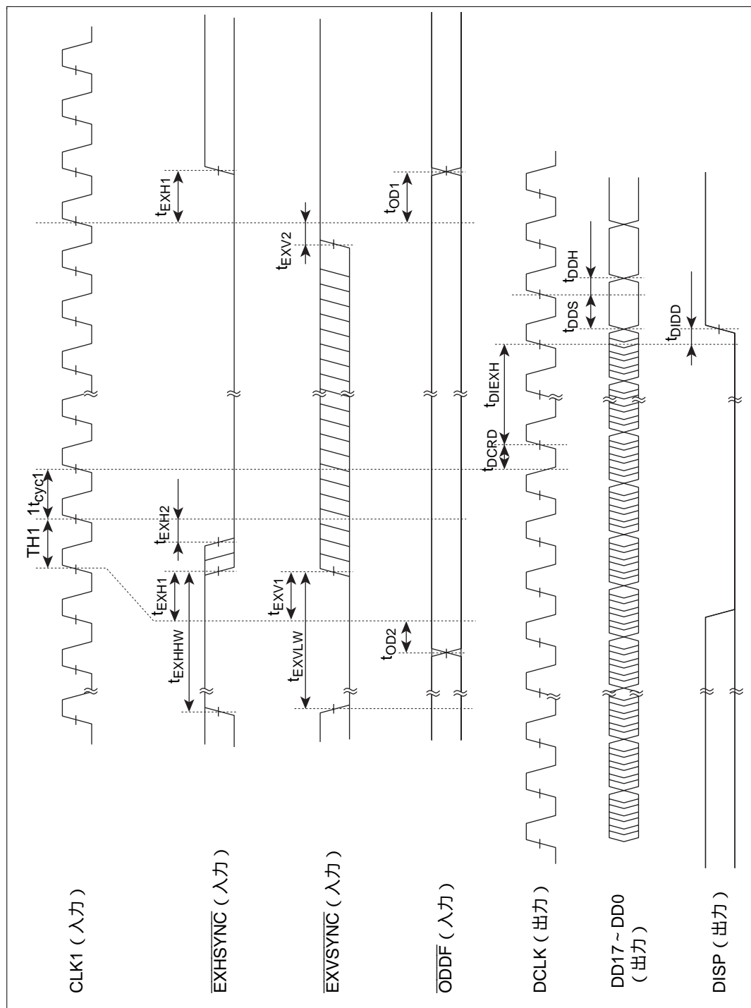
図 7.14 (4) TV 同期モード表示タイミング
