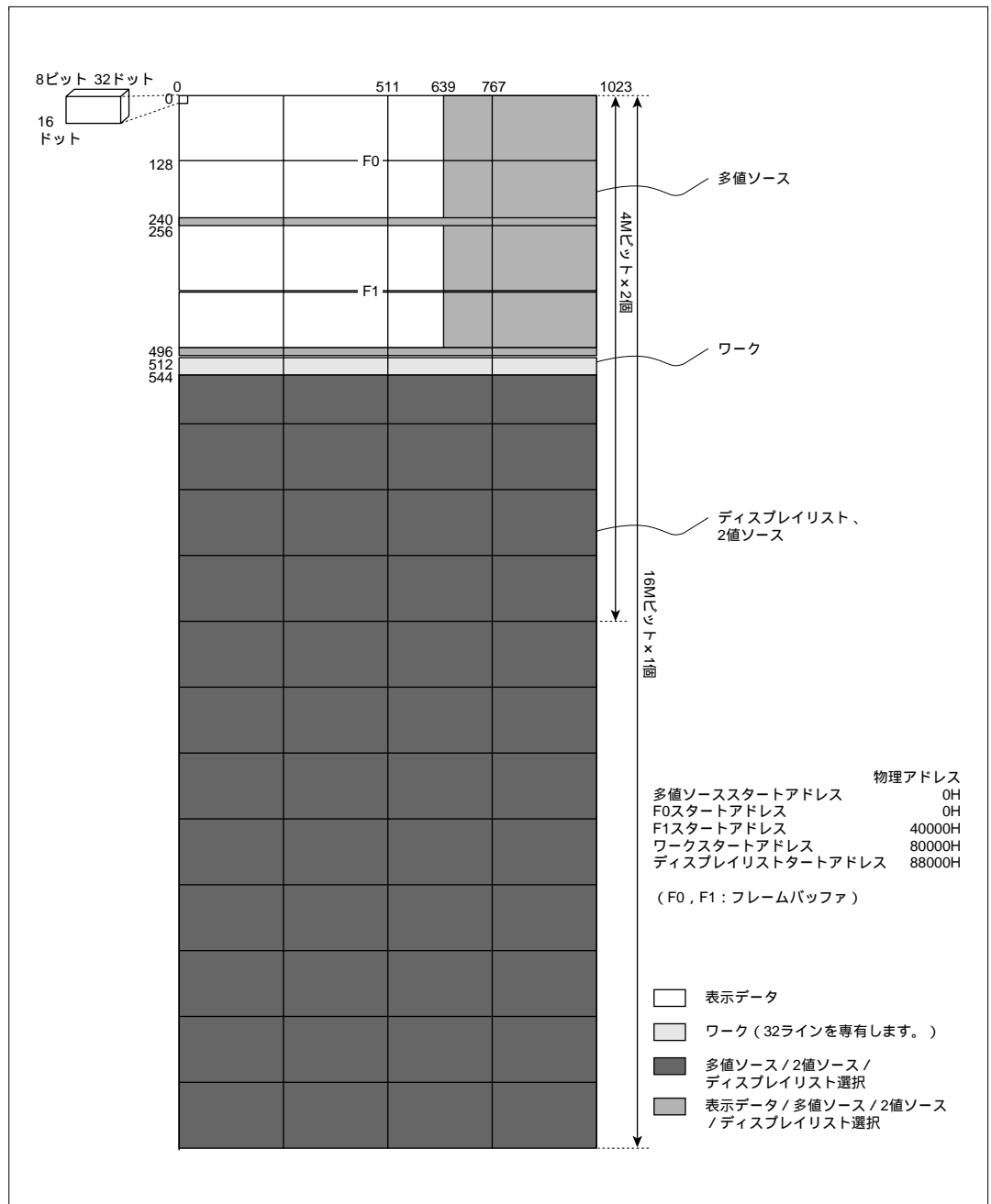
図 3.6 メモリマップ例 3 [ 8 ビット / 画素時 画面サイズ ( 640 × 240 相当時 ) ]
