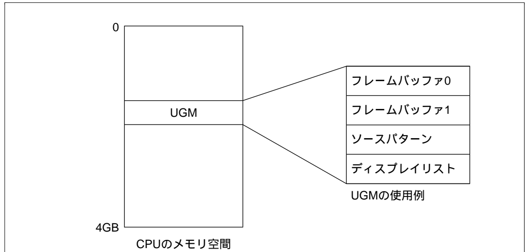
図 3.2 CPU メモリ空間に対する UGM のマッピング例
