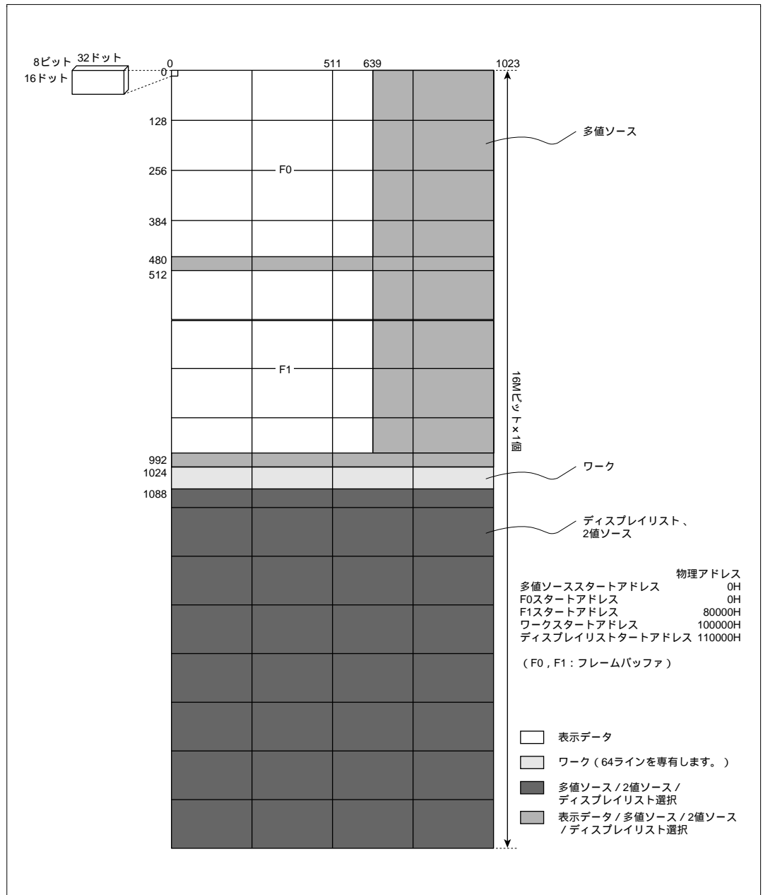
図 3.7 メモリマップ例 4 [8ビット/画素時 画面サイズ (640×480 相当時)]
