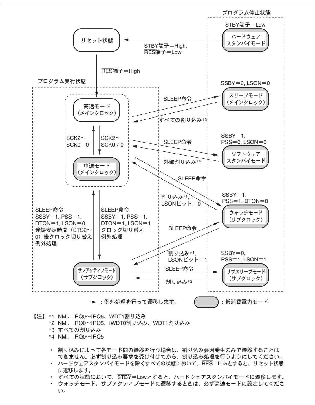
図 19.1 モード遷移図
