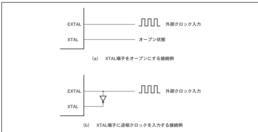
図 18.4 外部クロックの接続例
