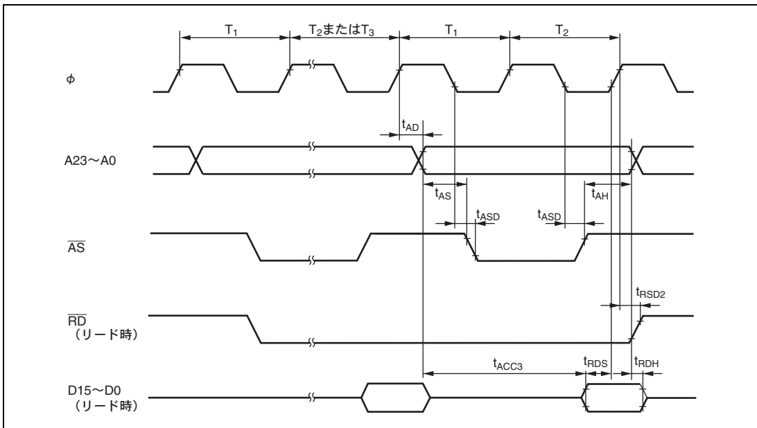
図 21.9 バースト ROM アクセスタイミング / 2 ステートアクセス
