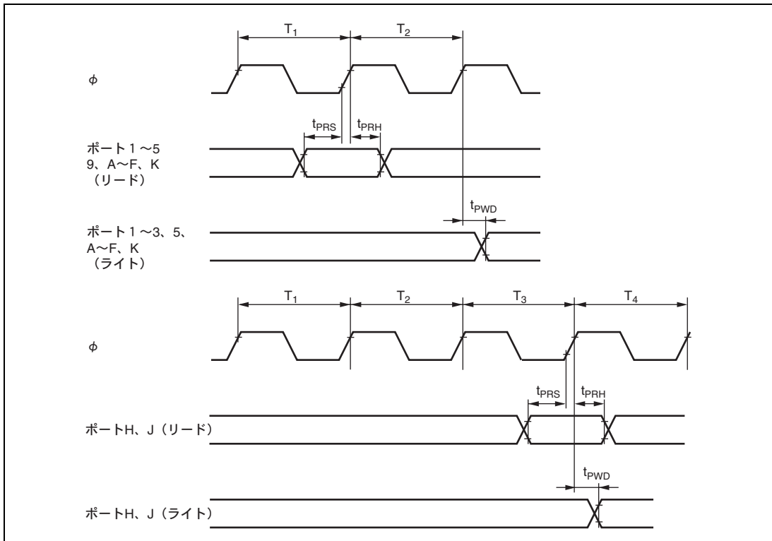
図 21.11 I/O ポート入出力タイミング
