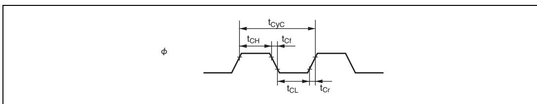
図 21.2 システムクロックタイミング
