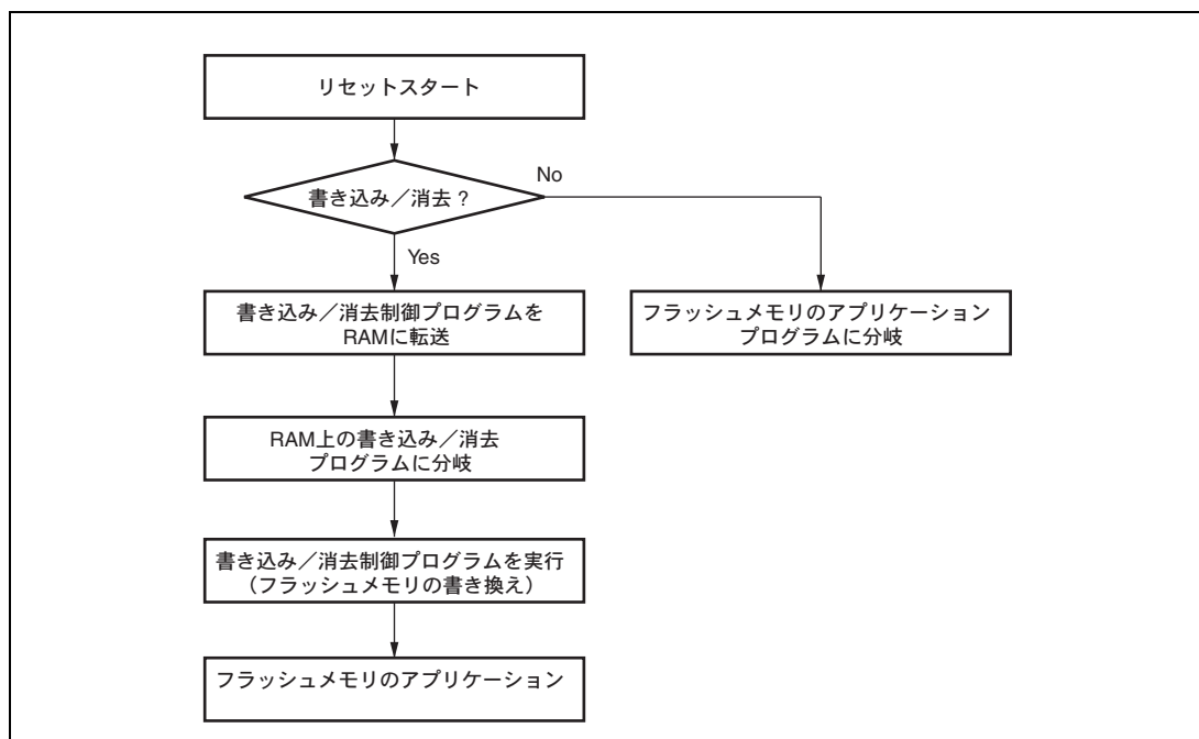
図 17.6 ユーザモードにおける書き込み/消去例
