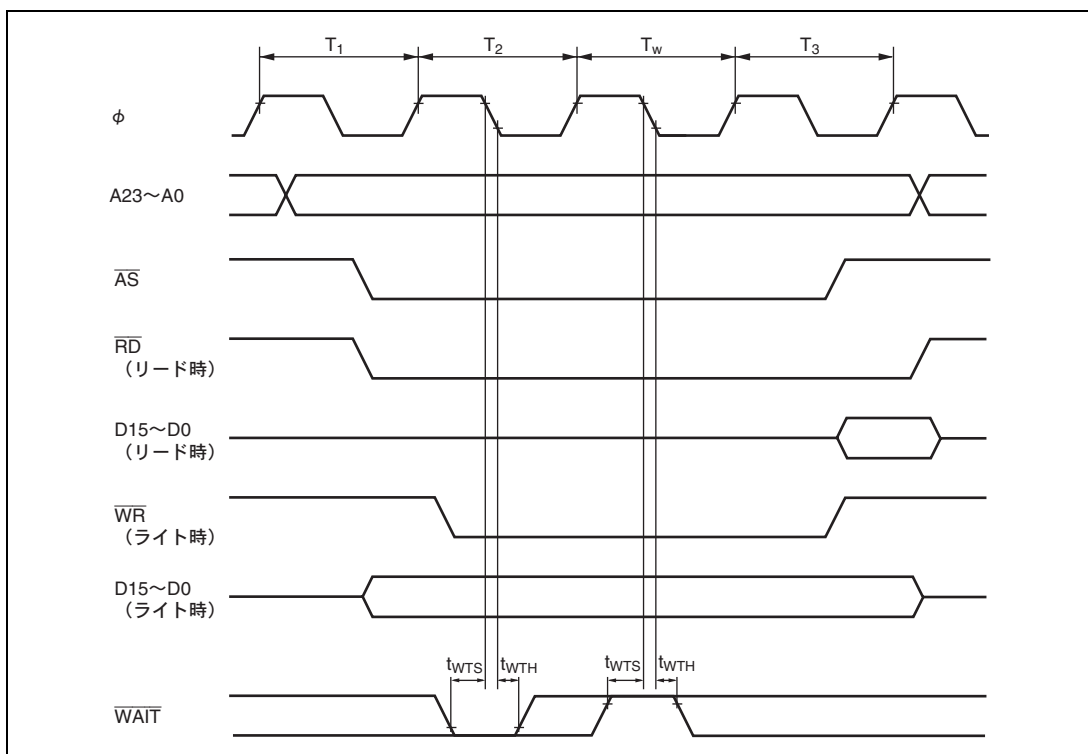
図 21.8 基本バスタイミング/3ステートアクセス1ウェイト
