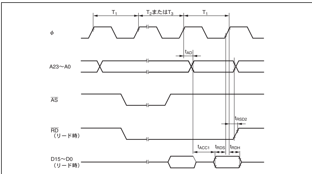
図 21.10 バースト ROM アクセスタイミング / 2 ステートアクセス
