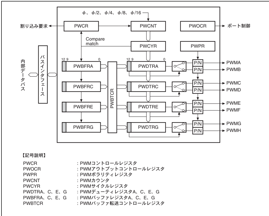
図 15.1 PWM のブロック図
