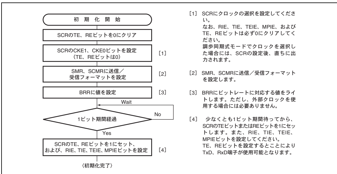
図 13.5 SCIの初期化フローチャートの例
