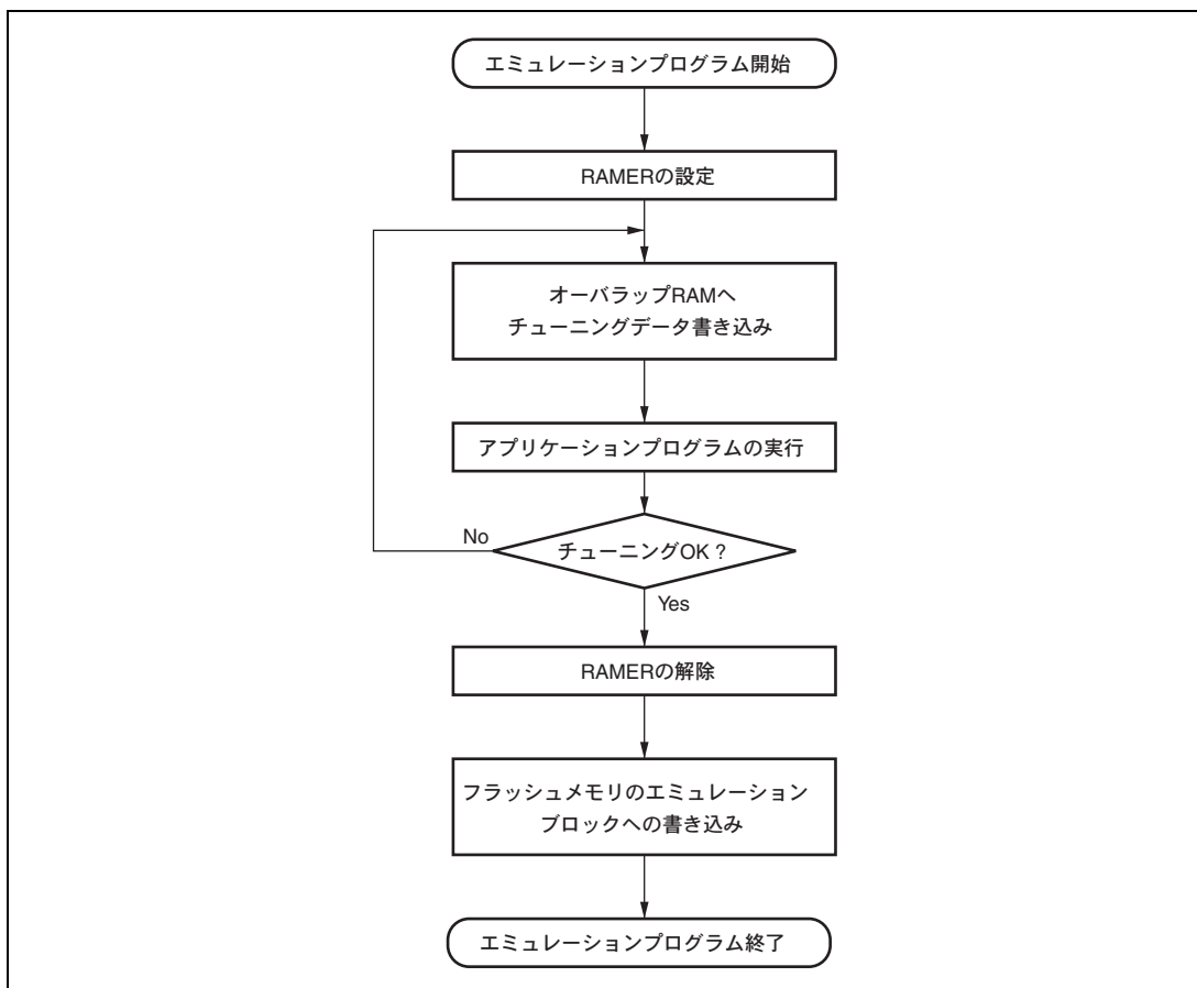
図 17.7 RAM によるエミュレーションフロー
