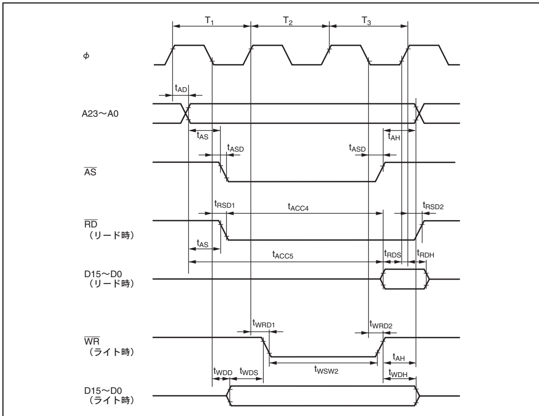
図 21.7 基本バスタイミング/3 ステートアクセス
