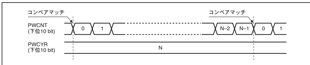
図 15.2 サイクルレジスタのコンペアマッチ
