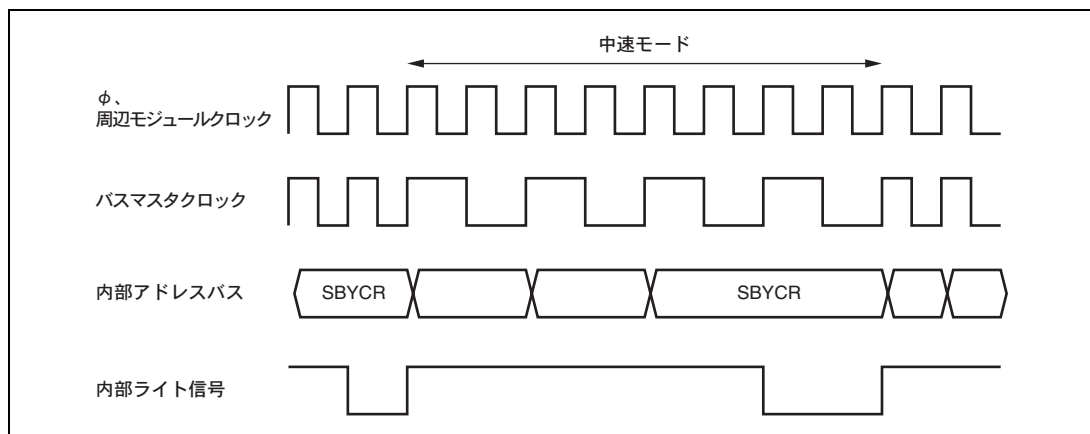
図 19.2 中速モードの遷移・解除タイミング
