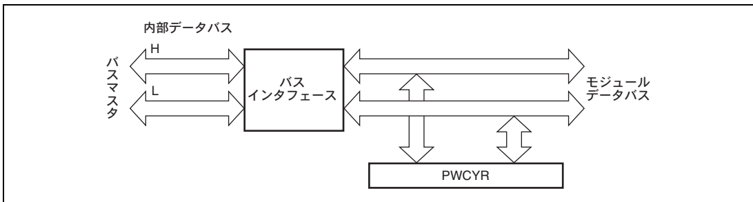
図 15.5 16 ビットレジスタのアクセス動作 (バスマスタ \leftrightarrow PWCYR (16 ビット))
