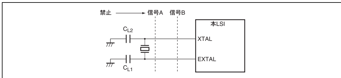
図 18.9 発振回路部のボード設計に関する注意事項
