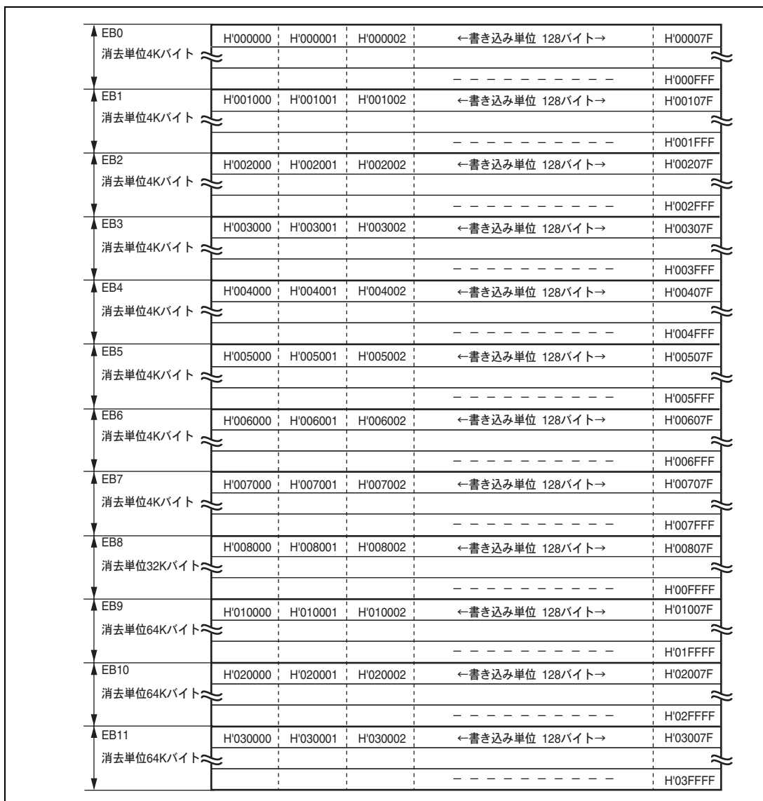
図 17.5 フラッシュメモリのブロック構成
