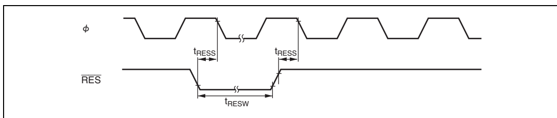
図 21.4 リセット入力タイミング
