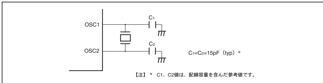
図 18.6 32.768kHz 水晶発振子の接続例
