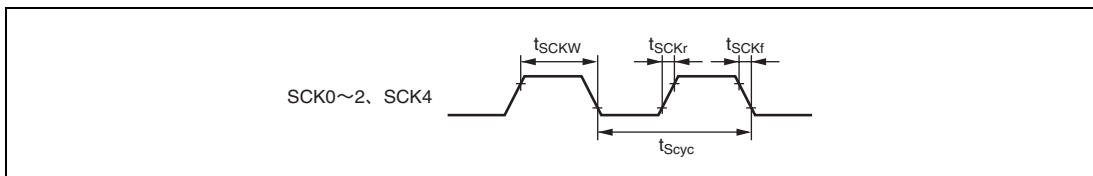
図 21.16 SCK クロック入力タイミング
