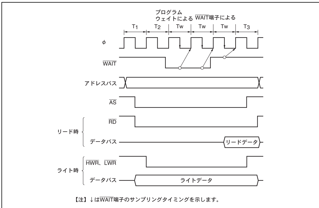
図 7.13 ウェイトステート挿入タイミング例
