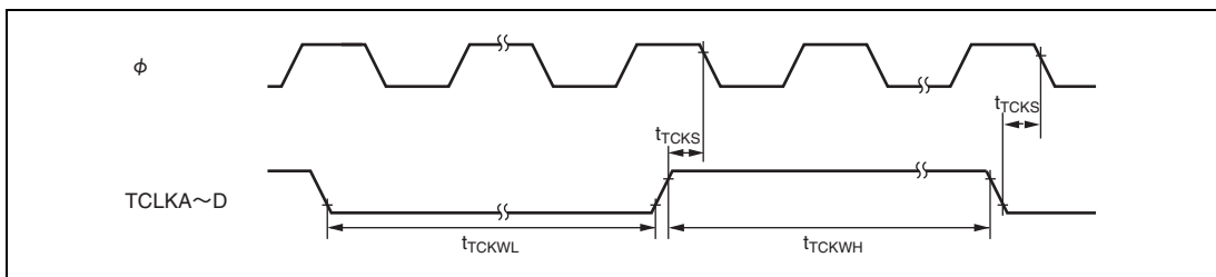
図 21.14 TPU クロック入力タイミング
