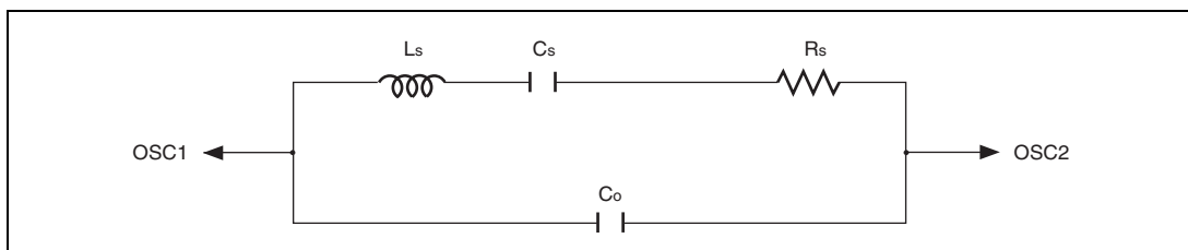
図 18.7 32.768kHz 水晶発振子の等価回路
