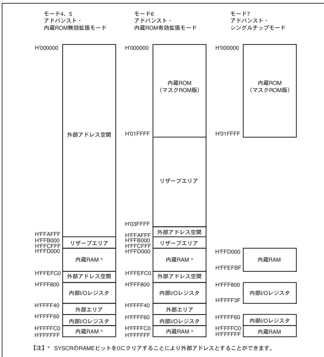
図 3.2 アドレスマップ (H8S/2608)
