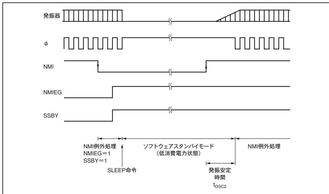
図 19.3 ソフトウェアスタンバイモードの応用例
