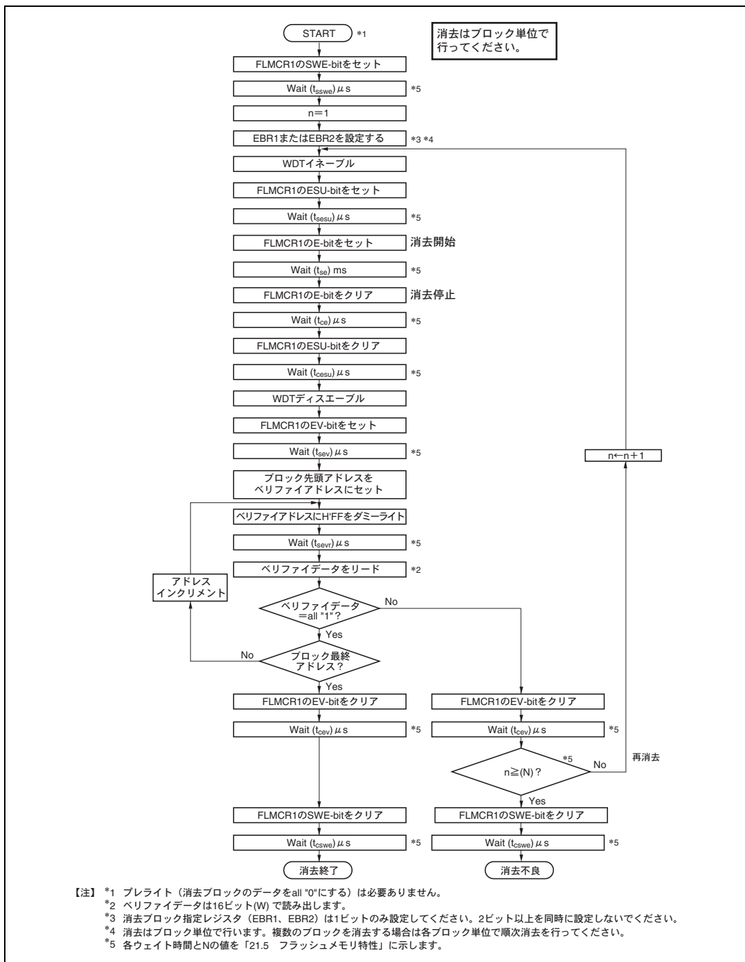
図 17.10 イレース/イレースペリファイフロー
