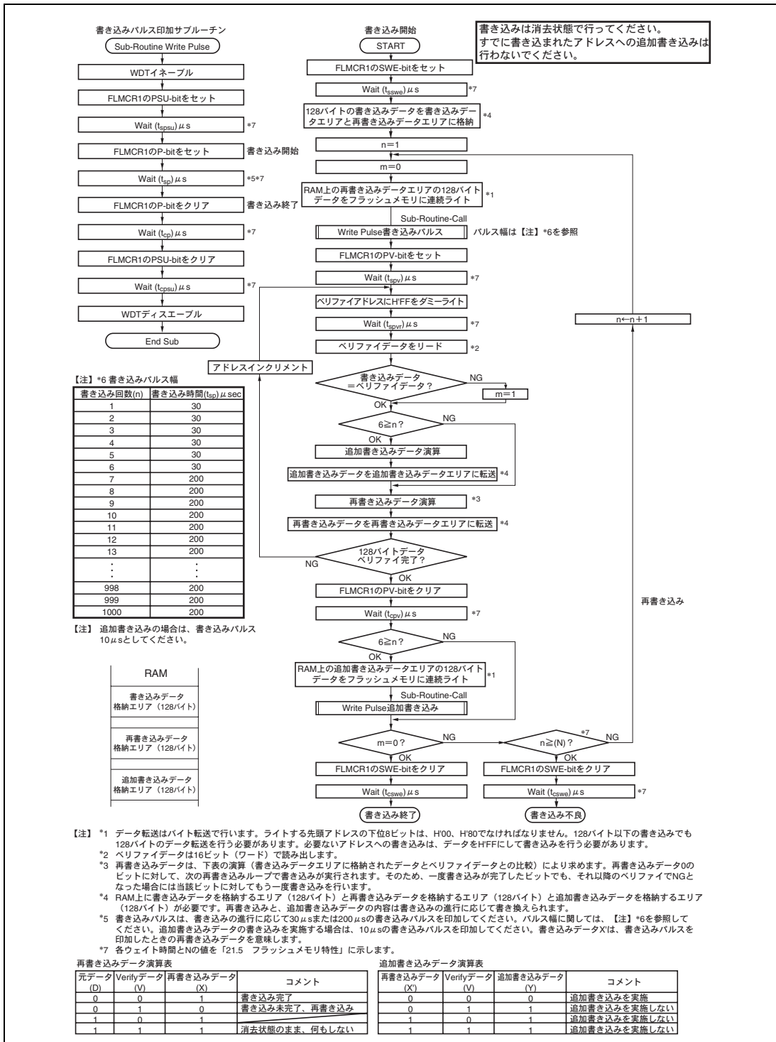
図 17.9 プログラム/プログラムペリファイフロー
