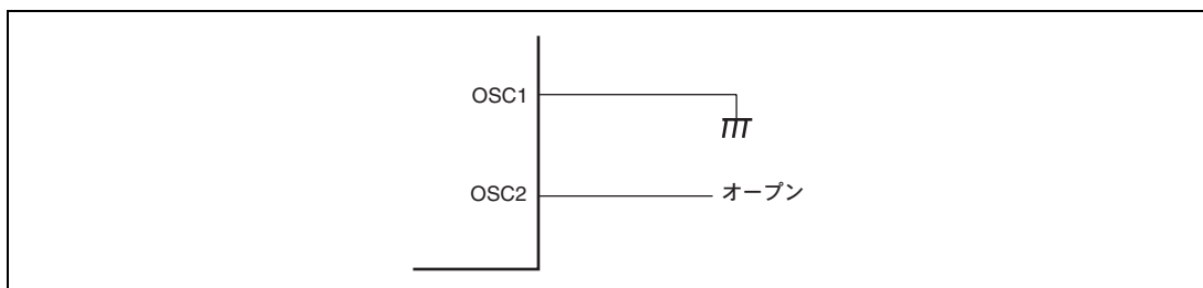
図 18.8 サブクロックを必要としない場合の端子処理
