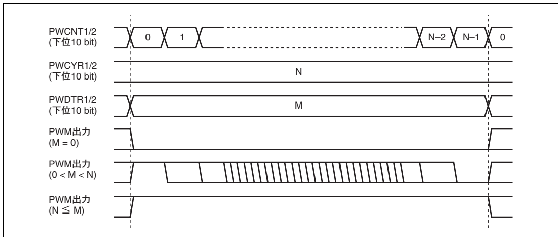
図 15.4 デューティレジスタの設定値による PWM 出力の相違 (PWPOR の OPS=0)
