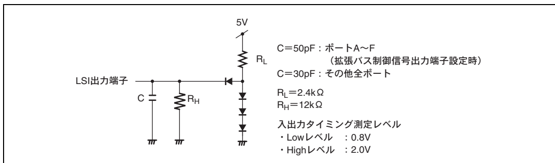
図 21.1 出力負荷回路
