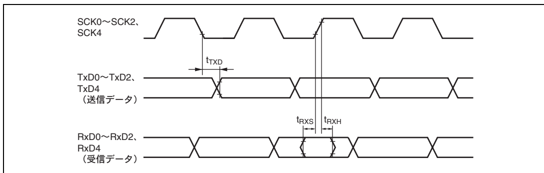
図 21.17 SCI 入出カタイミン／クロック同期式モード
