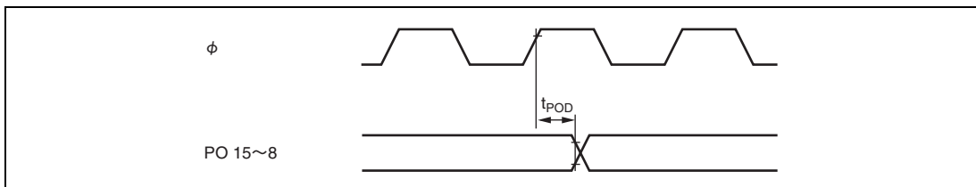
図 21.12 PPG 出カタイミン
