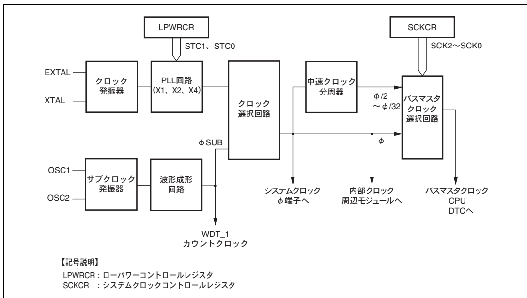
図 18.1 クロック発振器のブロック図
