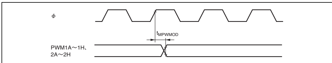
図 21.15 モータコントロール PWM 出力タイミング
