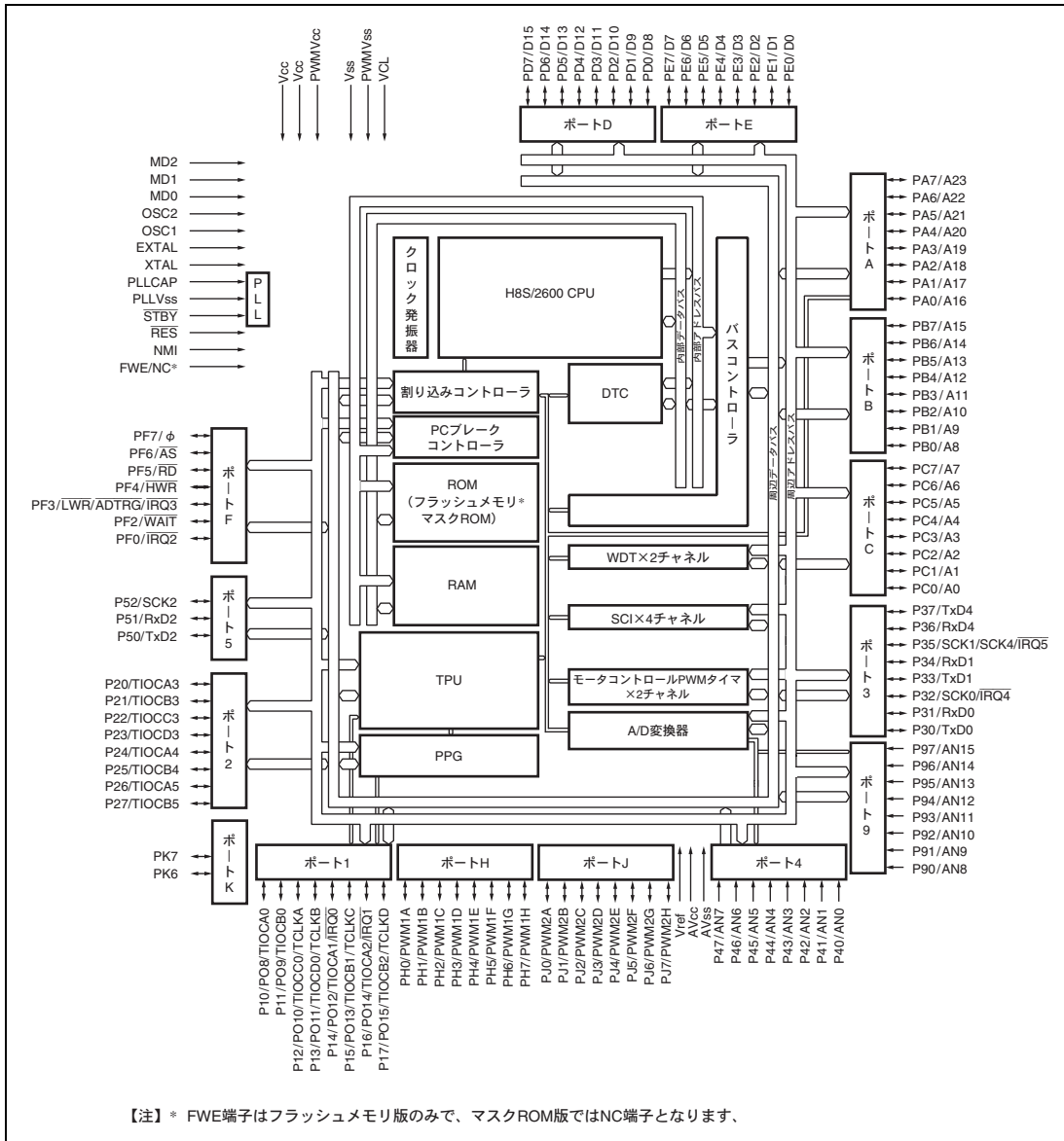
図 1.1 ブロック図
