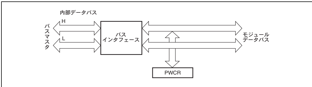
図 15.6 8 ビットレジスタのアクセス動作 (バスマスタ \leftrightarrow PWCR (上位 8 ビット))
