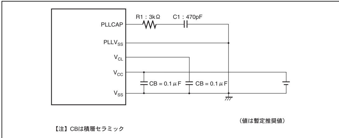
図 18.10 PLL 回路の外付け推奨回路
