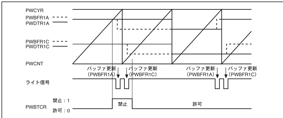
図 15.8 バッファ転送禁止動作説明
