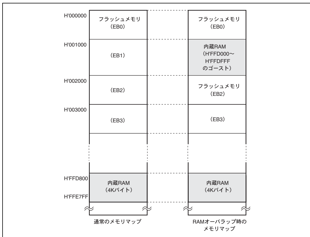
図 17.8 RAM のオーバーラップ例
