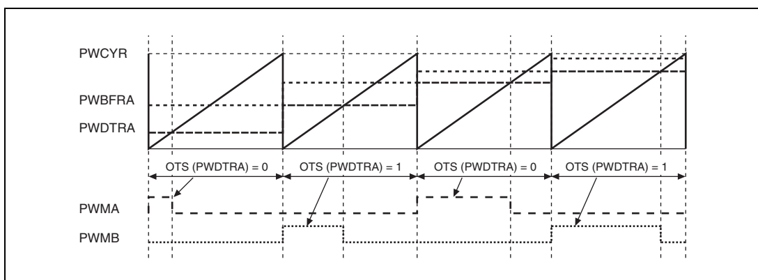
図 15.7 PWM の動作
