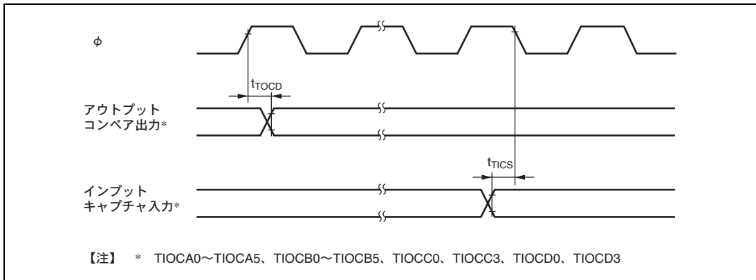
図 21.13 TPU 入出力タイミング
