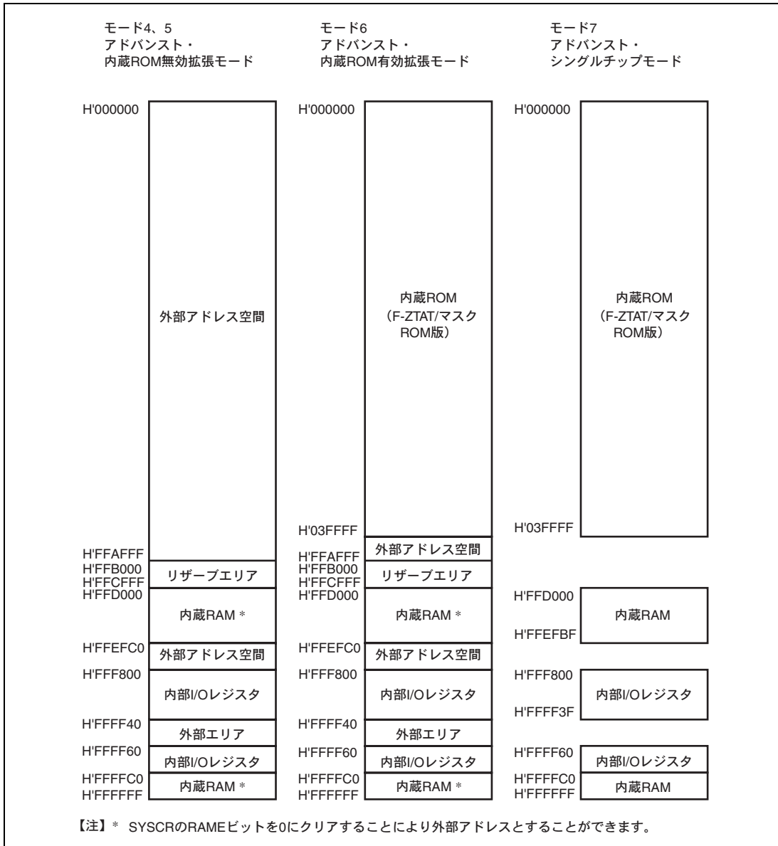
図 3.1 アドレスマップ (H8S/2609)
