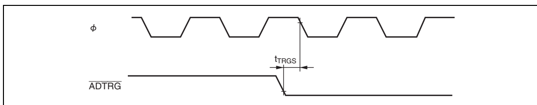
図 21.18 A/D 変換器外部トリガ入カタイミン
