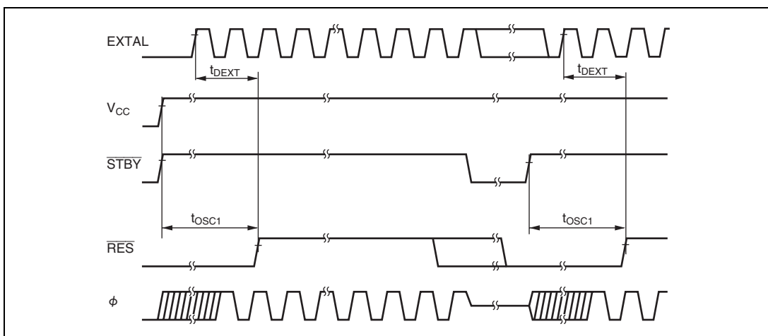
図 21.3 発振安定時間タイミング
