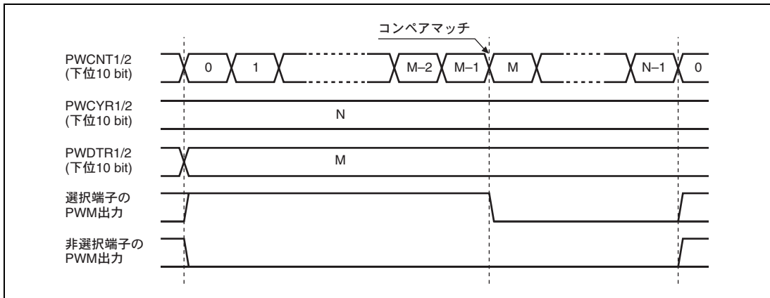
図 15.3 デューティレジスタのコンペアマッチ (PWPOR の OPS=0)
