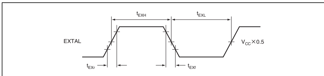
図 18.5 外部クロック入カタイミング
