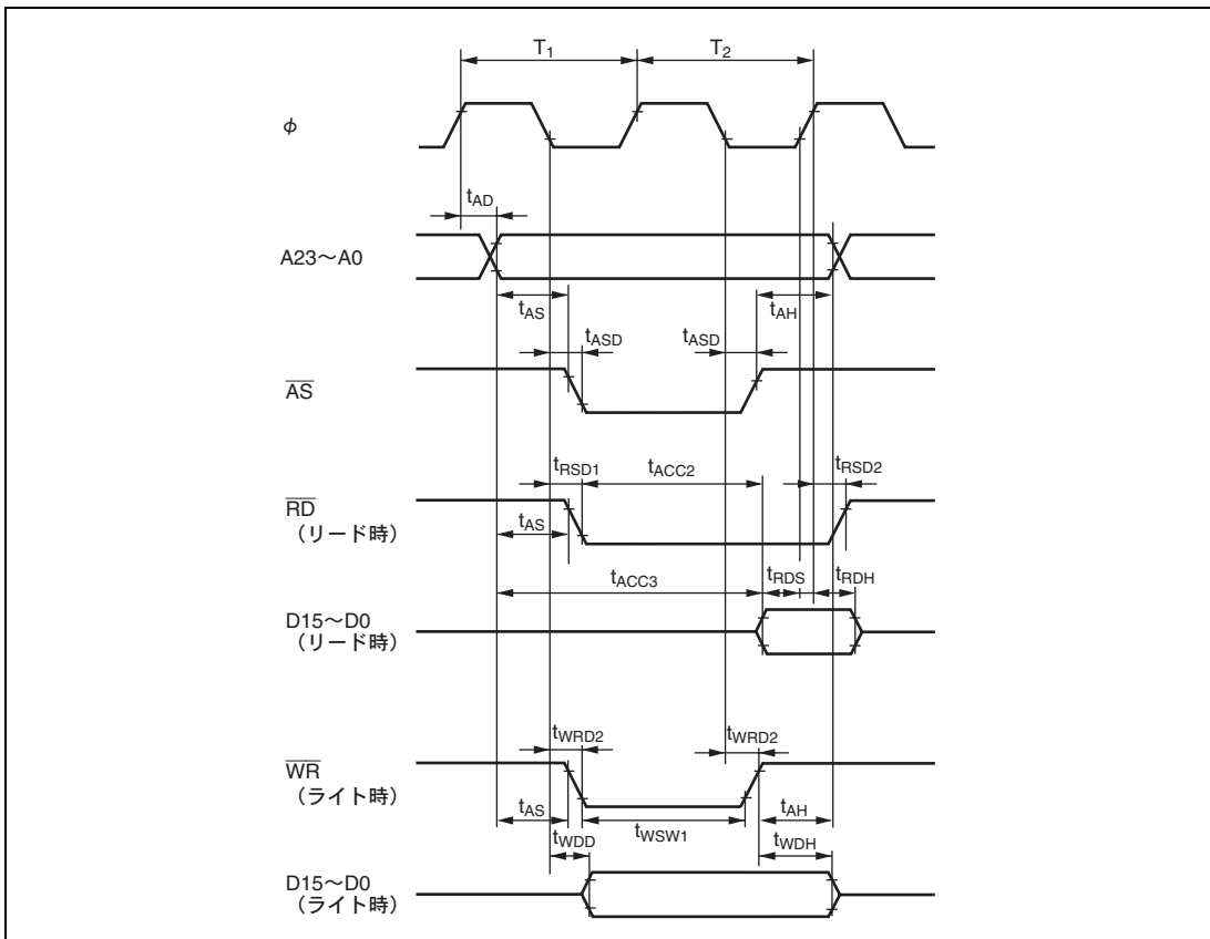
図 21.6 基本バスタイミング/2 ステートアクセス
