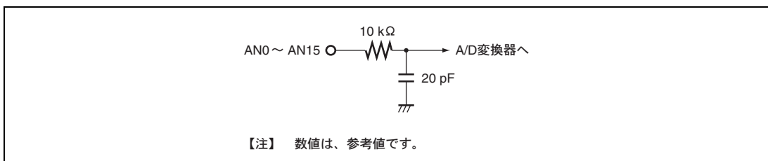
図 14.8 アナログ入力端子等価回路
