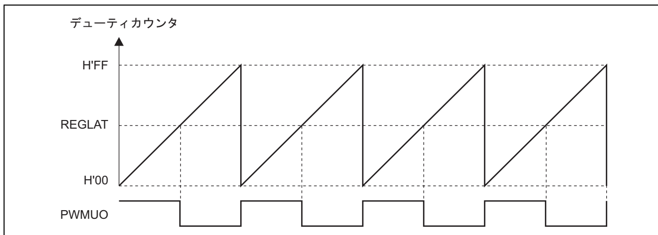
図 8.5 デューティカウンタの値と PWMU 出力のタイミング
