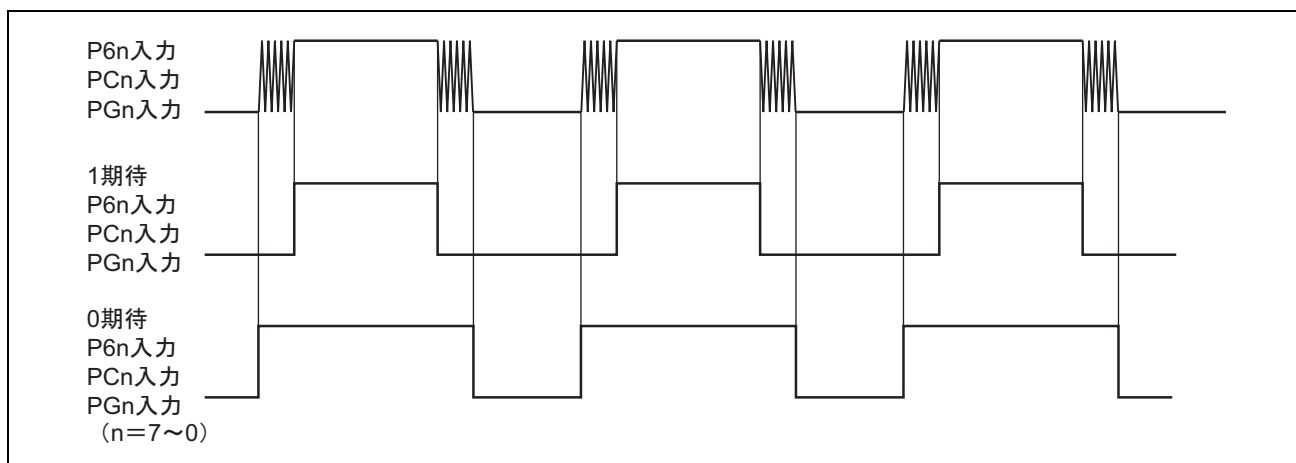
図 7.2 ノイズキャンセル動作概念図
