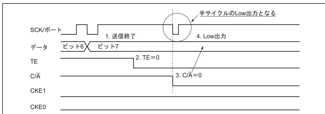
図 15.37 SCK 端子からポート端子へ切り替える時の動作
