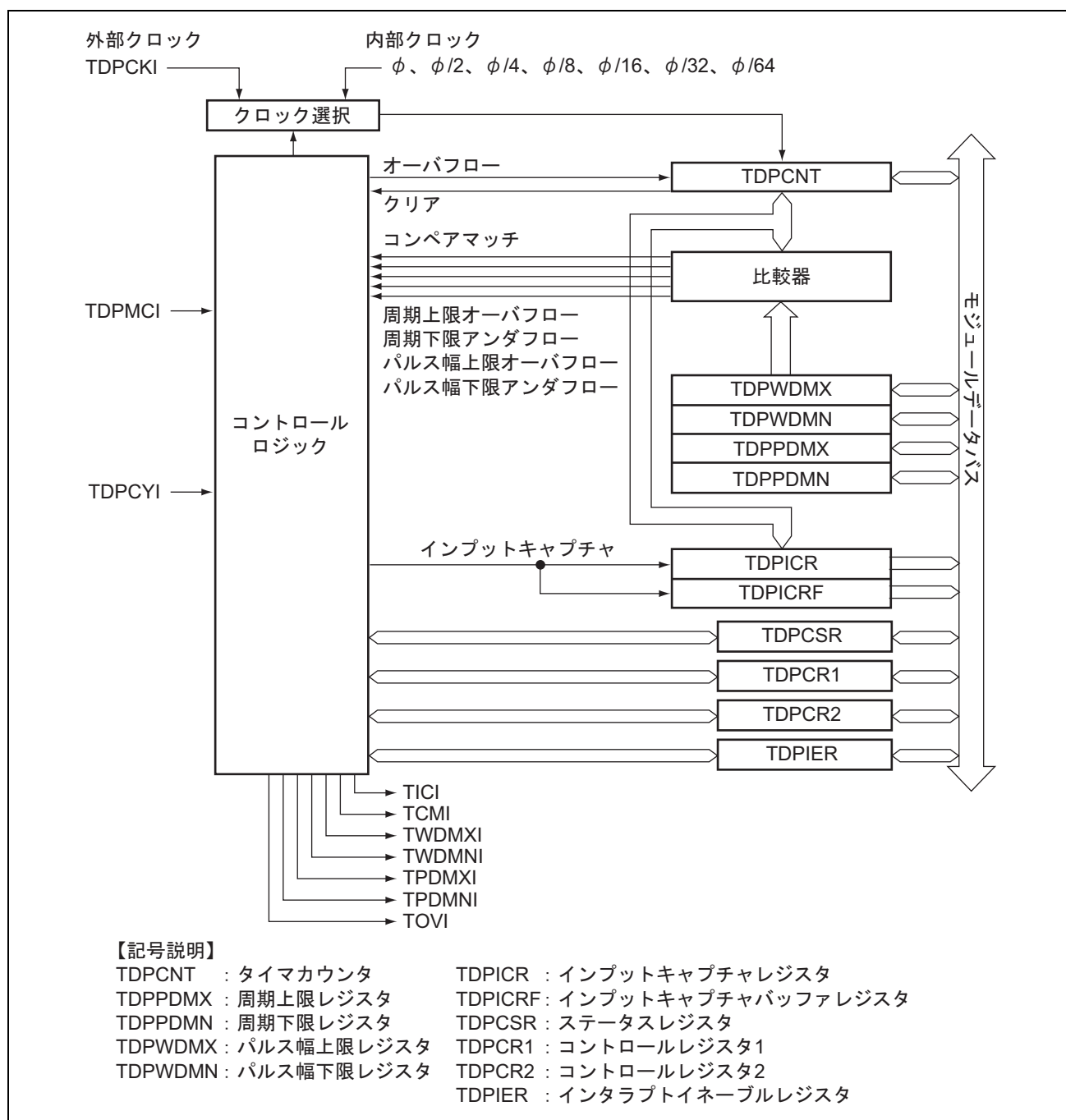
図 12.1 TDP ブロック図
