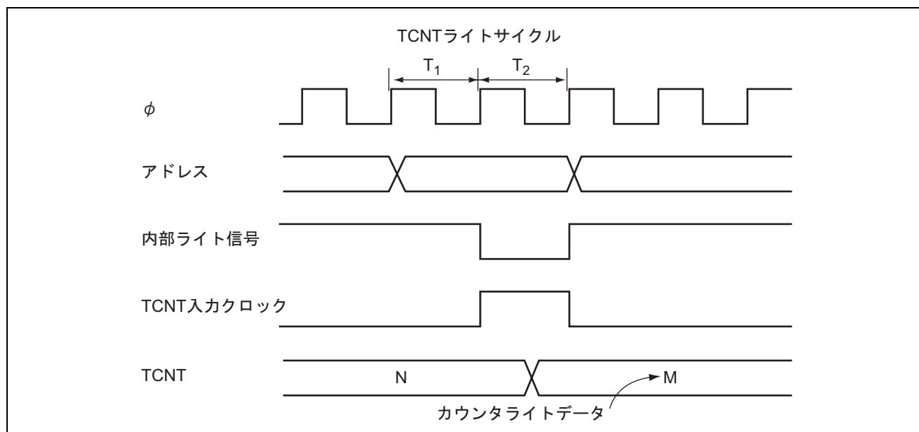
図 14.6 TCNT のライトとカウントアップの競合
