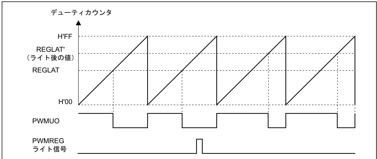
図 8.6 PWMREG を変更した場合の PWMU 出力波形
