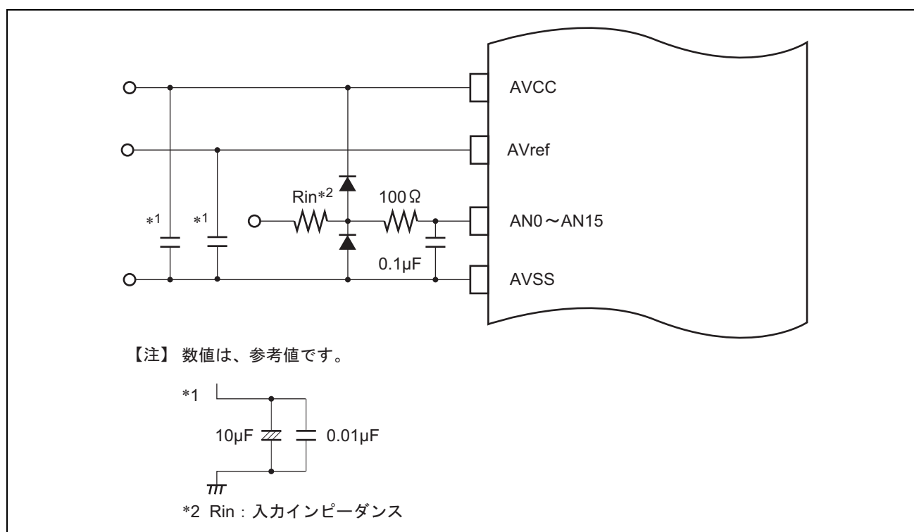
図 20.6 アナログ入力保護回路の例
