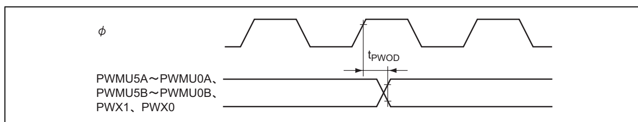
図 26.19 PWMU、PWMX 出力タイミング
