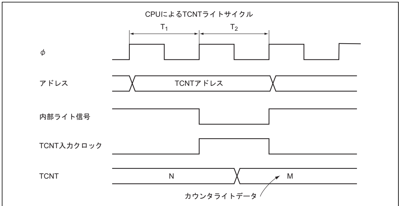
図 13.14 TCNT のライトとカウントアップの競合
