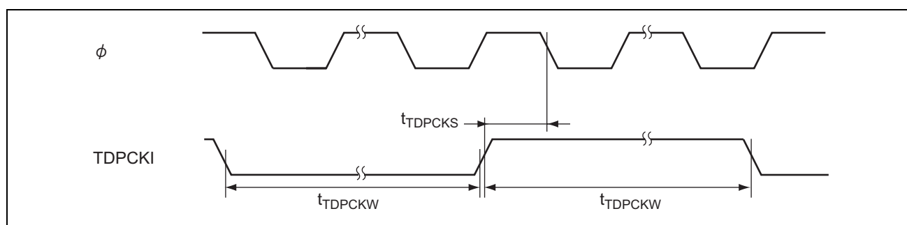
図 26.18 TDP クロック入力タイミング
