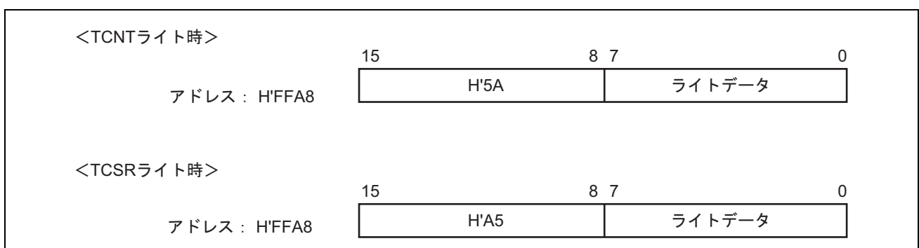
図 14.5 TCNT、TCSR へのライト (WDT_0 の例)
