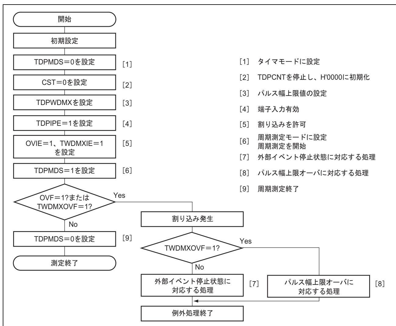
図 12.12 周期測定モード設定例 (パルス幅上限値を設定する場合)
