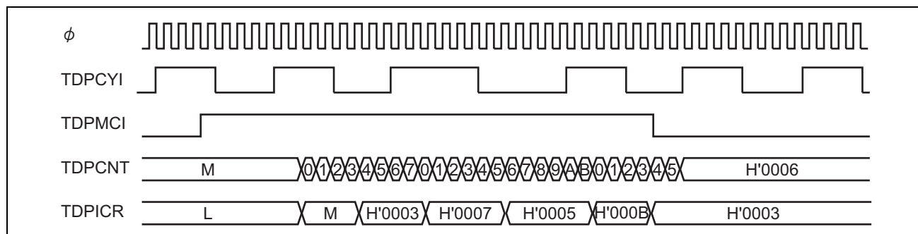
図 12.9 CMMS ビットが 1 にセットされているときの周期測定のタイミング例
