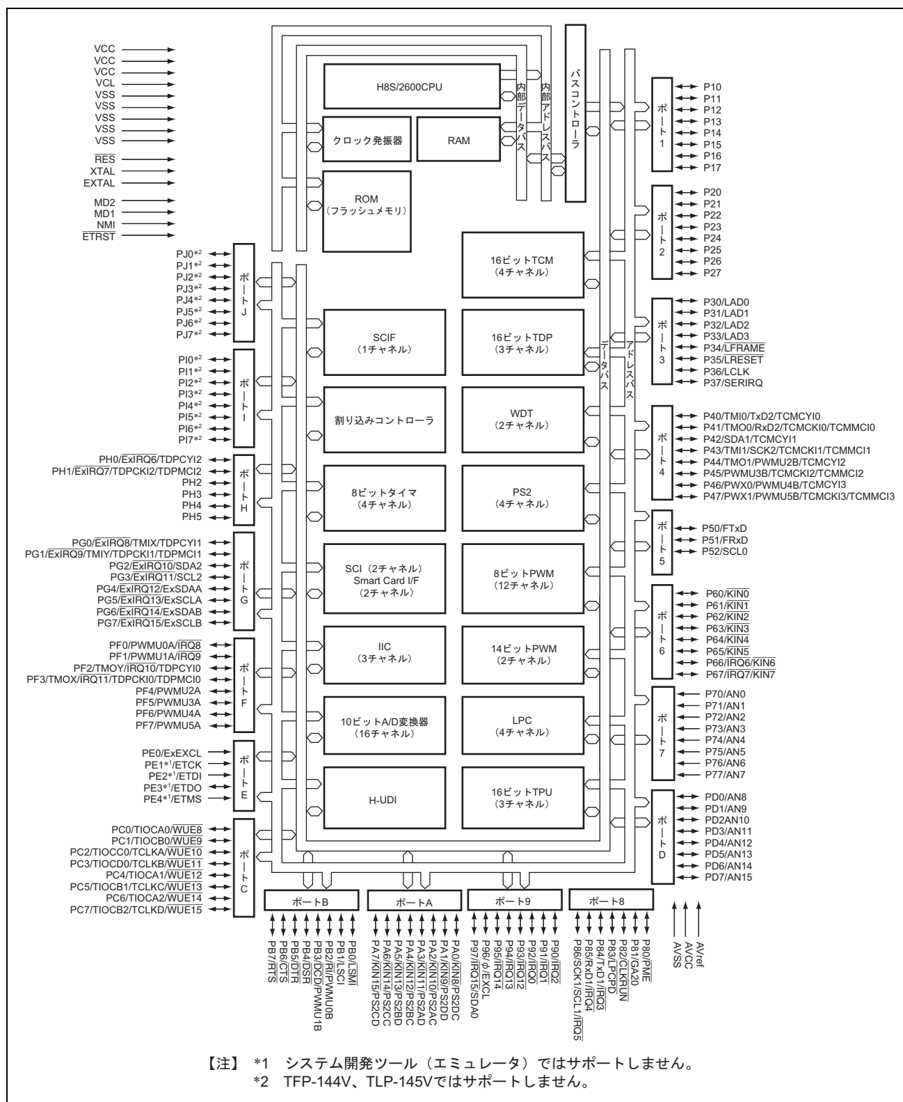
図 1.2 ブロック図
