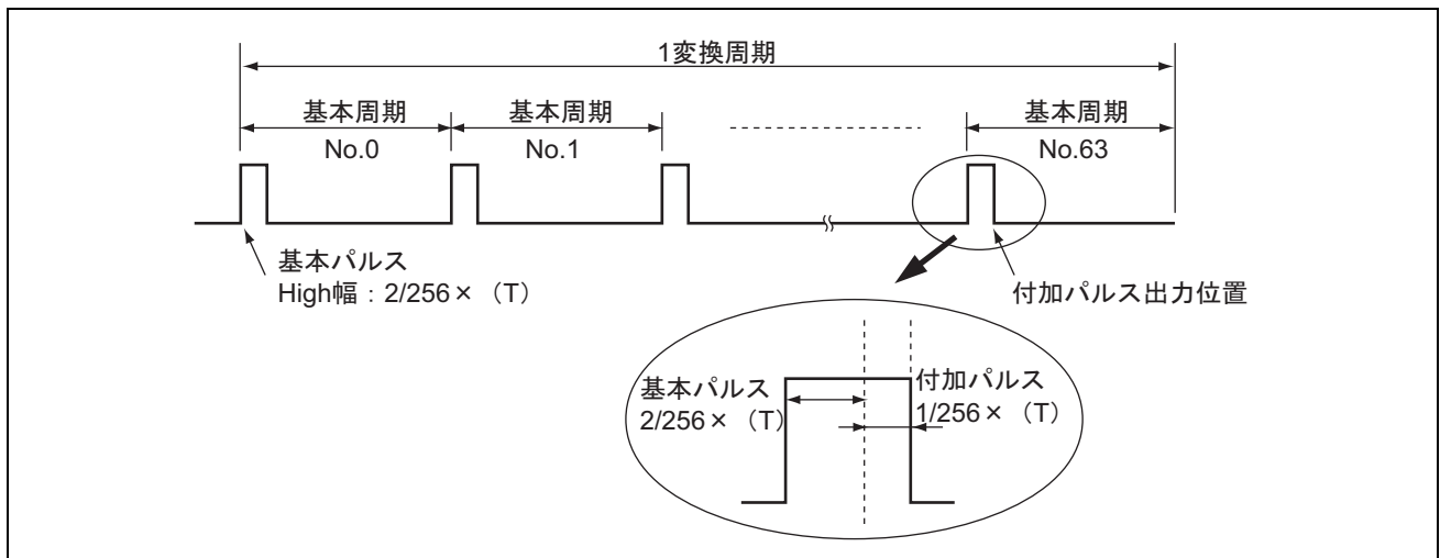
図 9.7 DADR = H'0207 のときの出力波形 (OS = 1)
