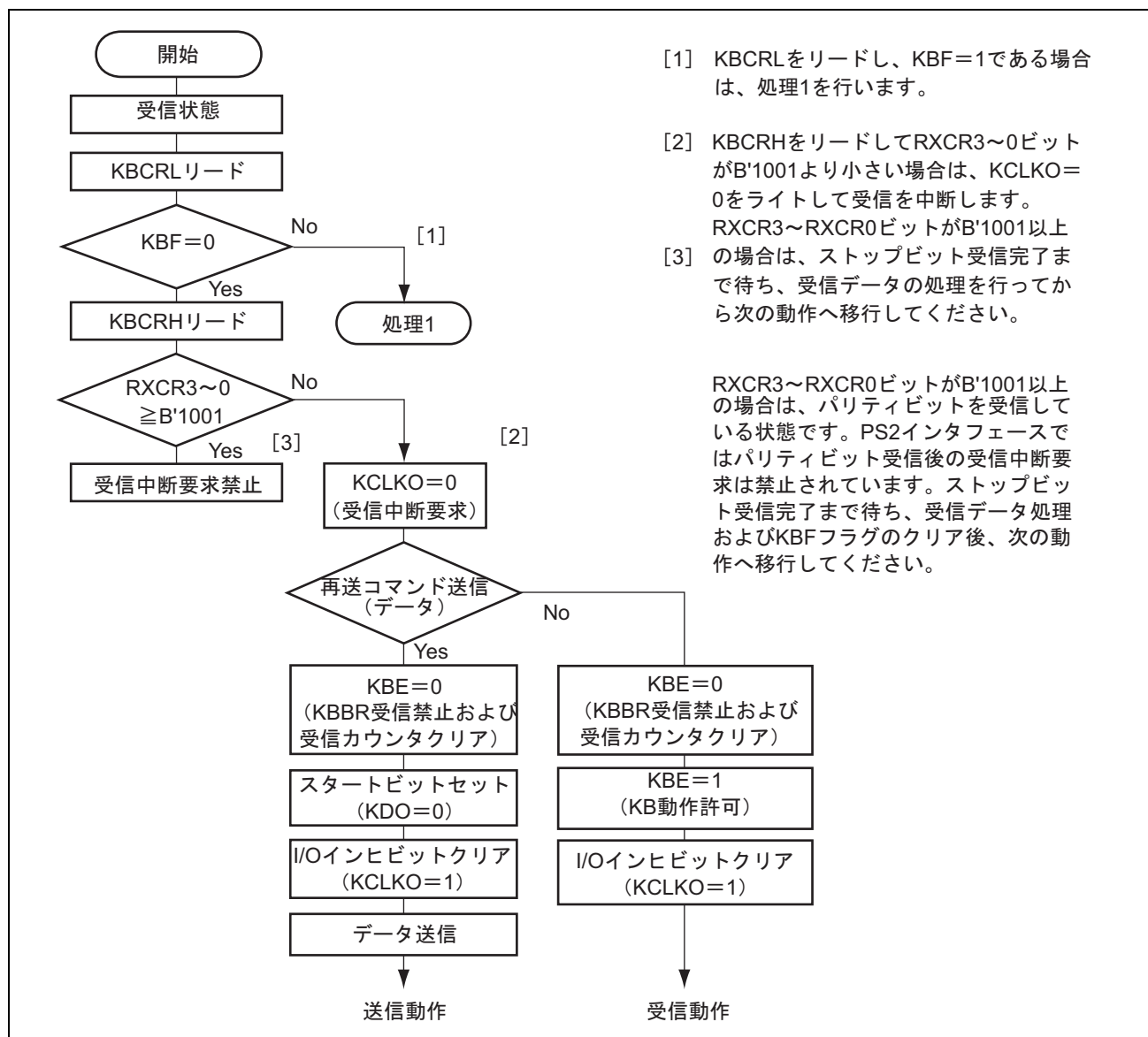
図 18.7 受信中断処理フローチャートの例 (1)
