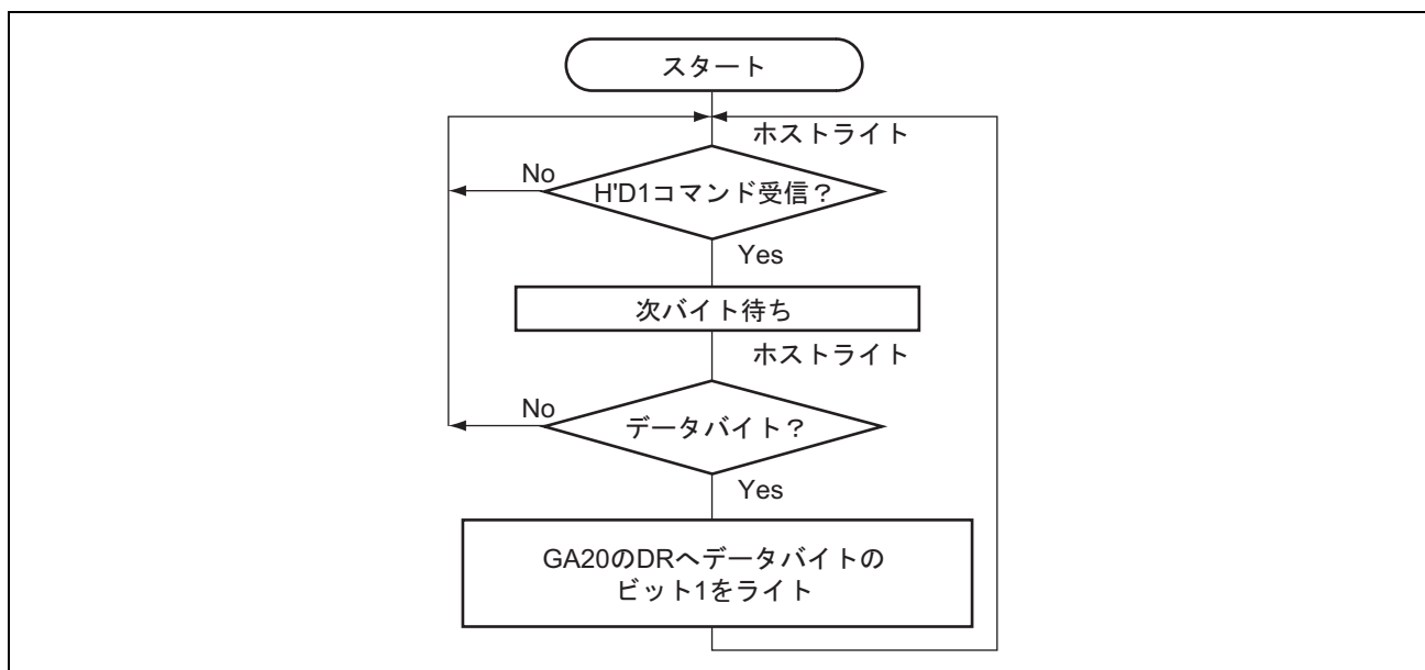
図 19.4 GA20 出力
