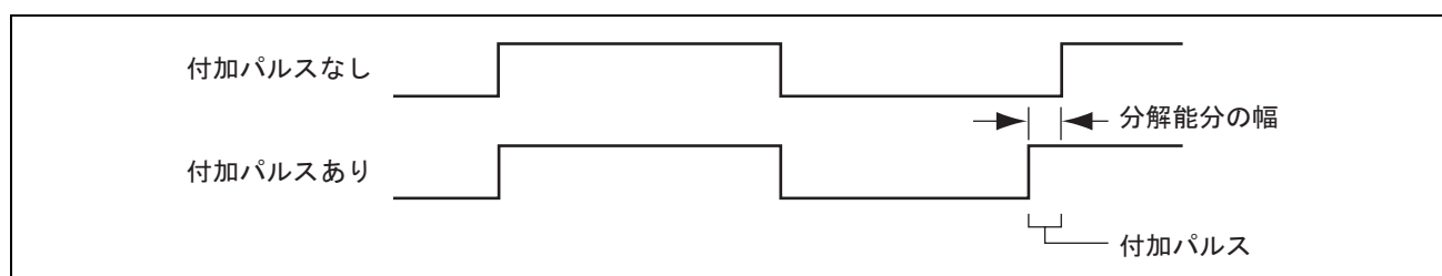
図 8.8 付加パルスタイミング例 (PWMREG 上位 4 ビットが B'1000)
