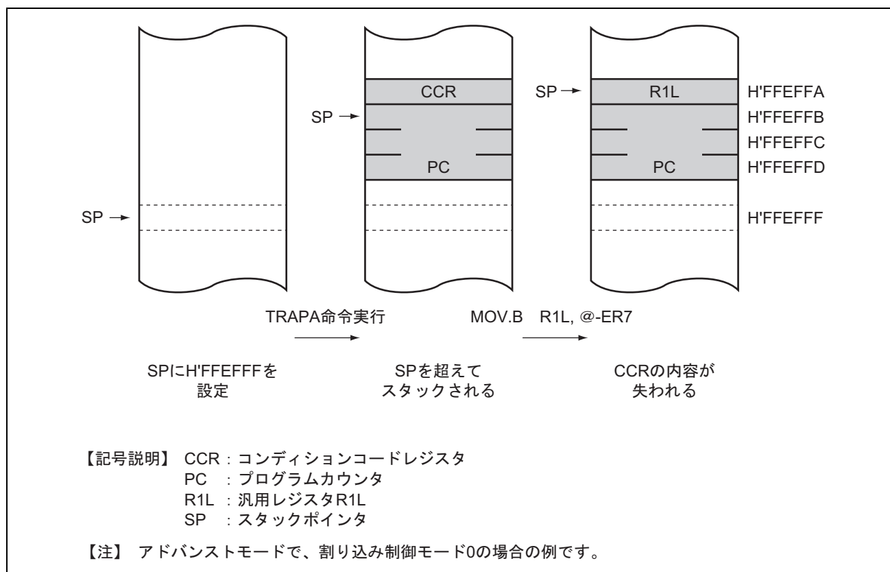
図 4.3 SP を奇数に設定したときの動作
