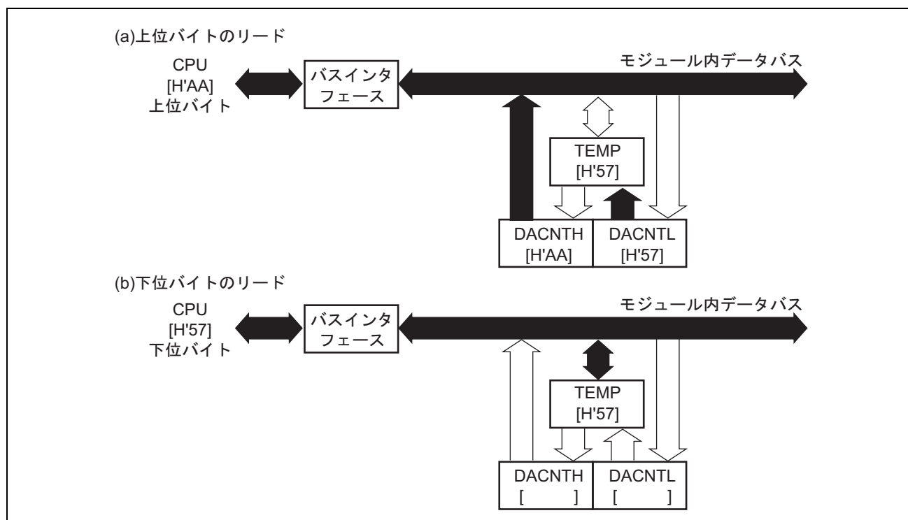
図 9.2 DACNT のアクセス動作 (2) (DACNT→CPU[H'AA57]リード時)
