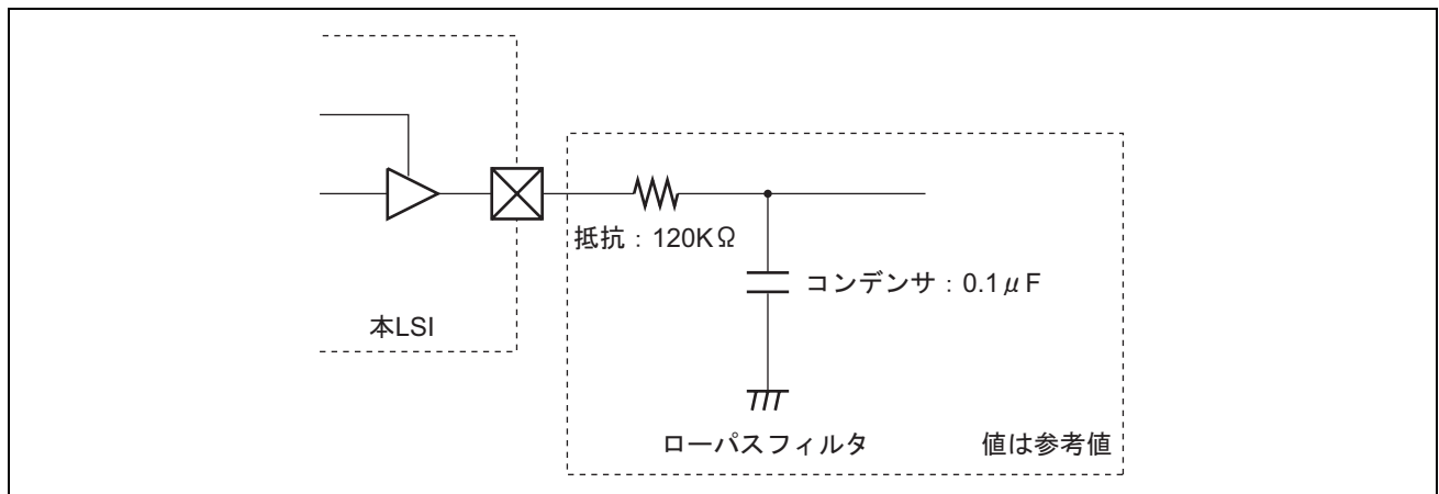
図 8.10 D/A として使用する場合の回路例
