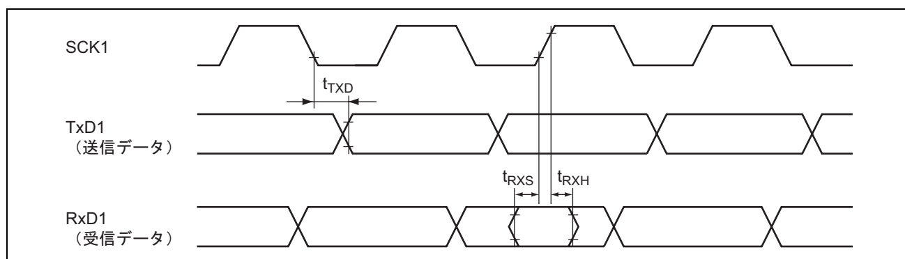
図 26.21 SCI 入出力タイミング/クロック同期式モード
