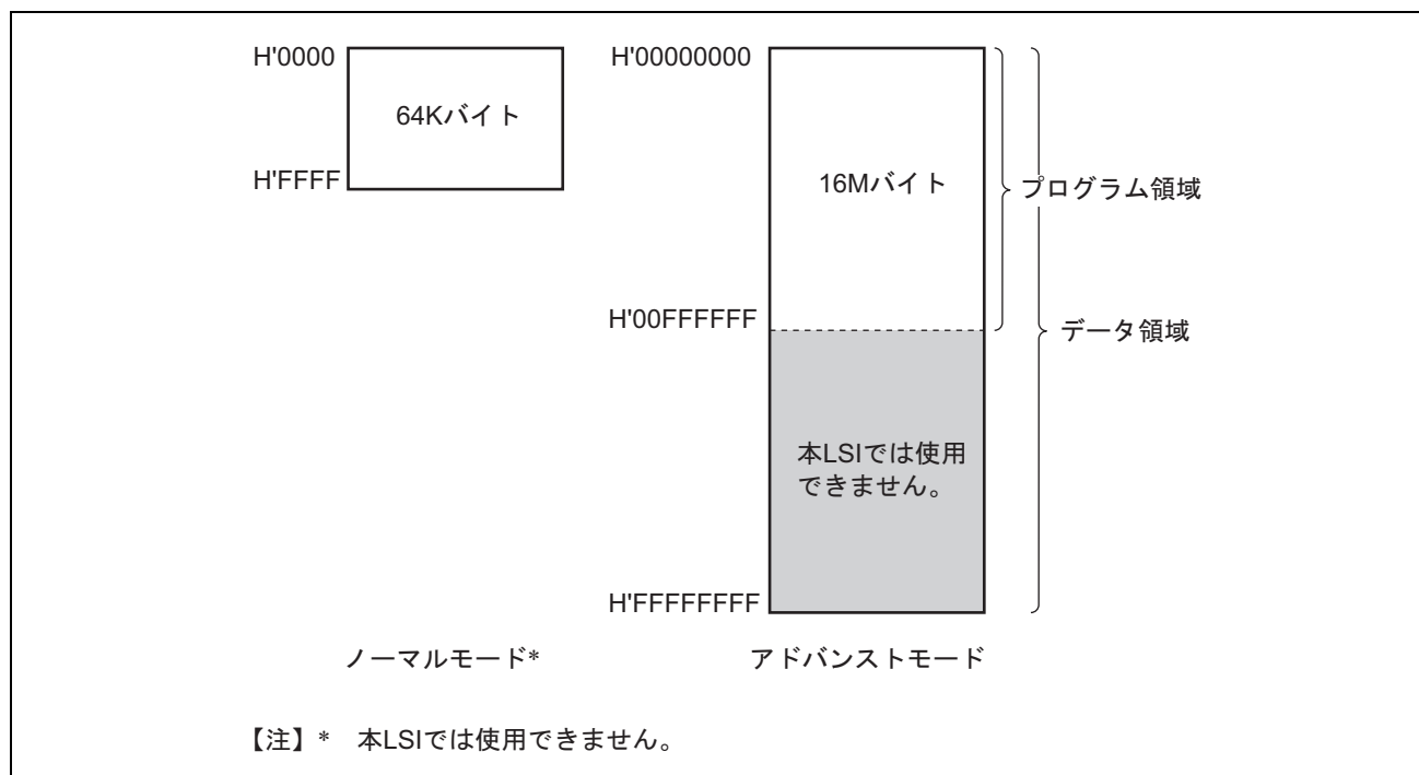
図 2.5 アドレス空間
