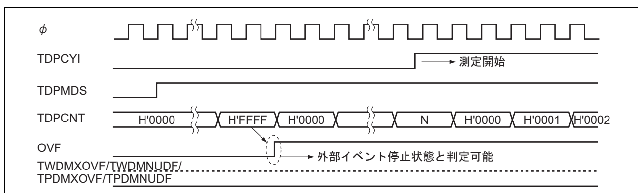
図 12.10 外部イベント停止状態のタイミング例 (1)
