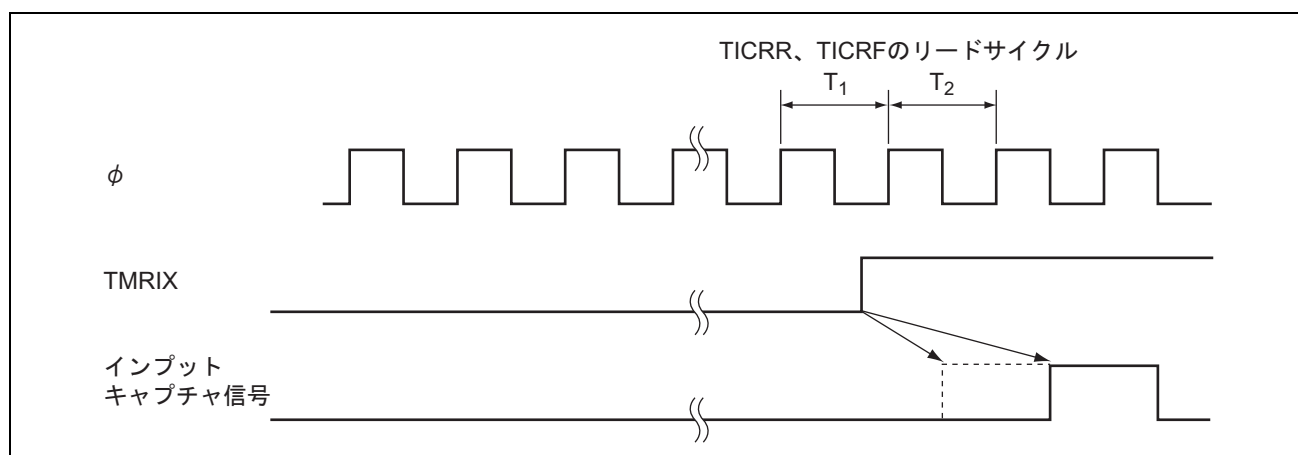
図 13.12 インพุットキャプチャ信号タイミング (TICRR、TICRF のリード時に、インพุットキャプチャ入力を入力した場合)
