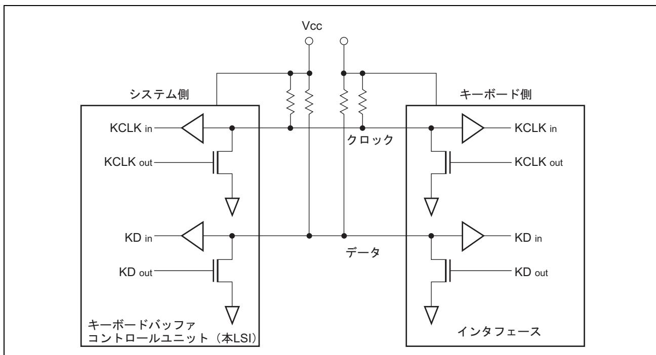
図 18.2 PS2 接続方法
