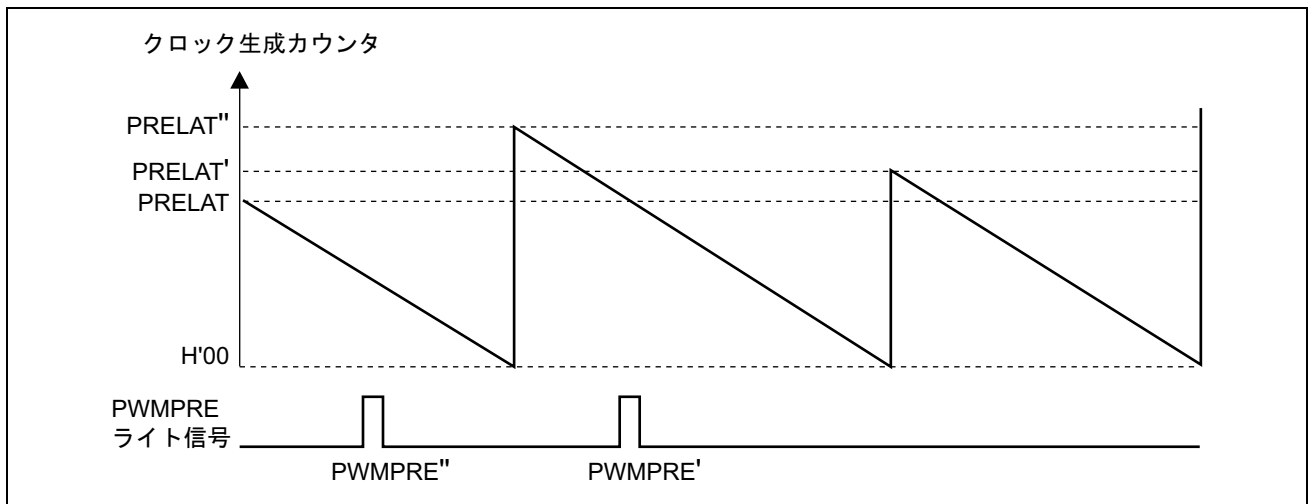
図 8.7 PWMPRE を変更した場合の PRELAT 更新タイミング
