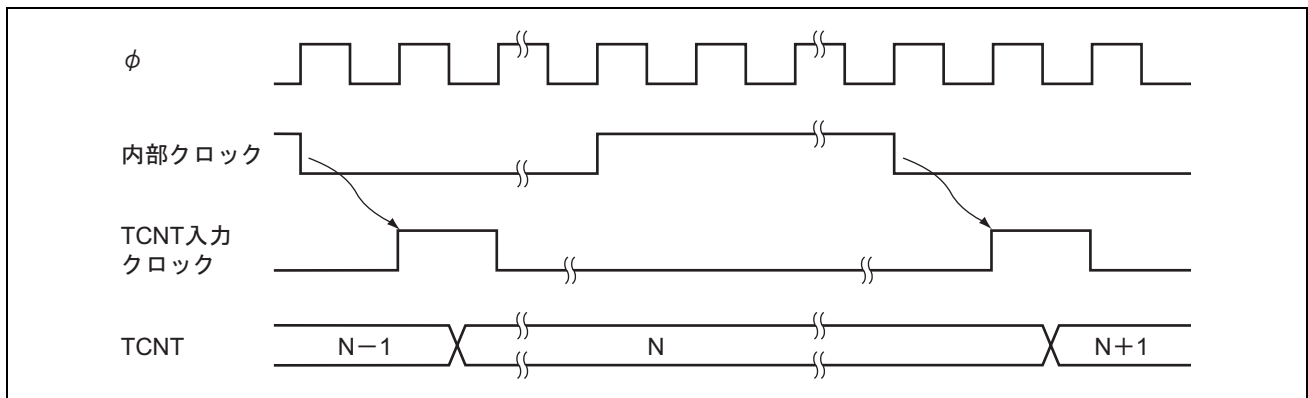
図 13.4 内部クロック動作時のカウントタイミング
