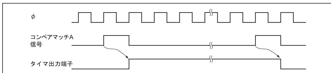
図 13.7 コンペアマッチ A 信号によるトグル出力のタイマ出力タイミング
