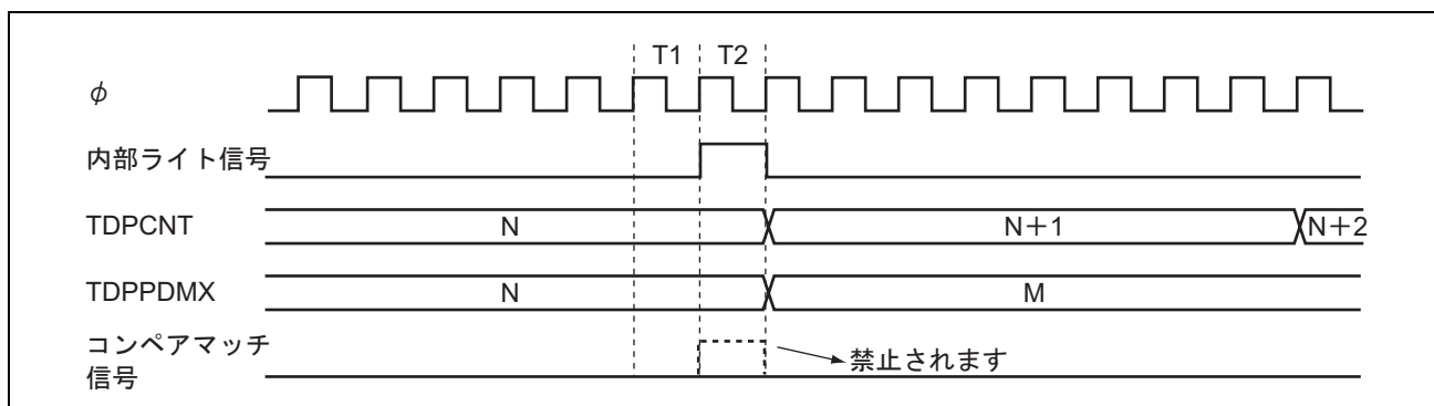
図 12.14 TDPPDMX のライトとコンペアマッチの競合
