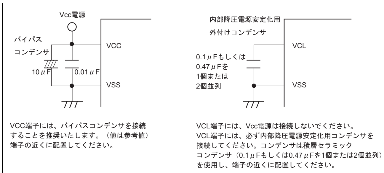
図 26.29 VCC 端子と VCL 端子のコンデンサ接続方法
