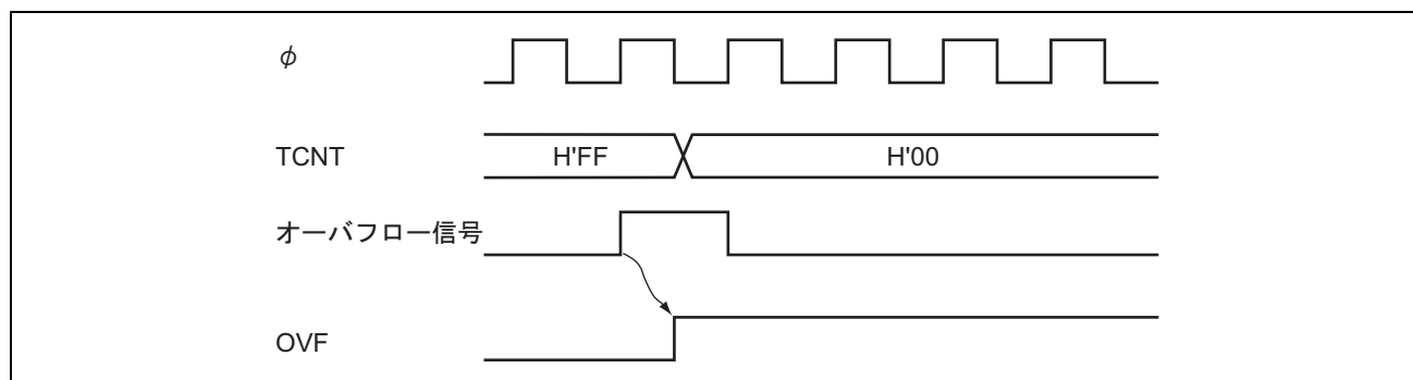
図 13.10 OVF フラグのセットタイミング
