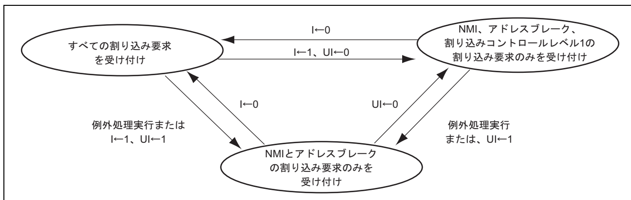
図 5.8 割り込み制御モード 1 の状態遷移
