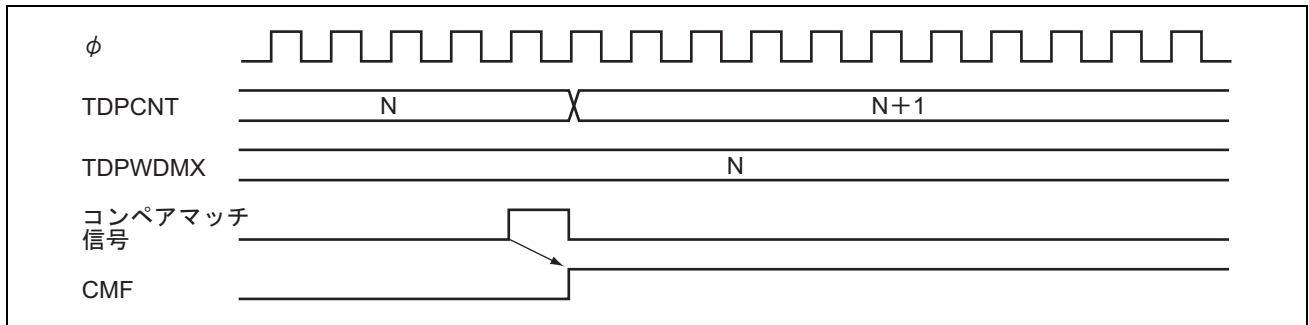
図 12.6 コンペアマッチ時の CMF フラグのセットタイミング
