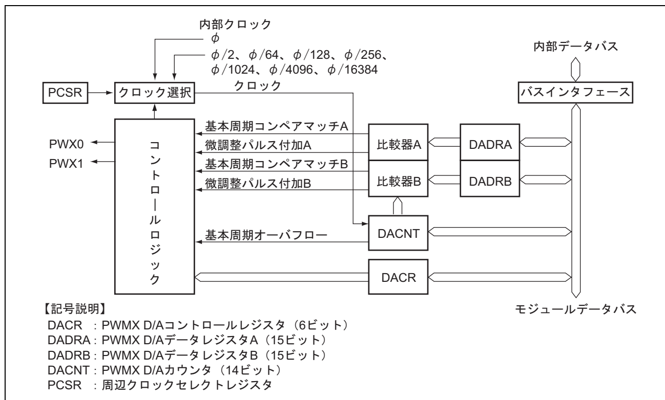
図 9.1 PWMX ( D/A ) のブロック図
