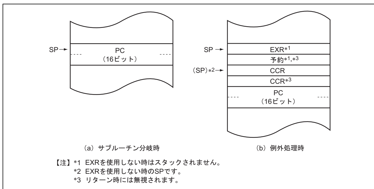
図 2.2 ノーマルモードのスタック構造
