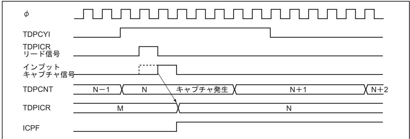
図 12.15 インพุットキャプチャと TDPICR リードの競合
