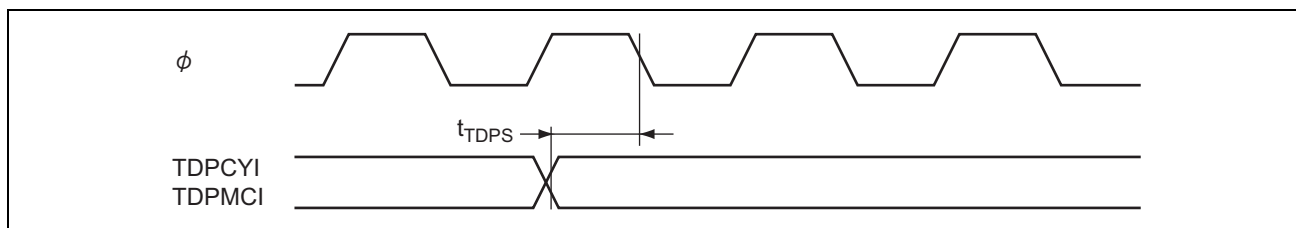
図 26.17 TDP 入力セットアップ時間
