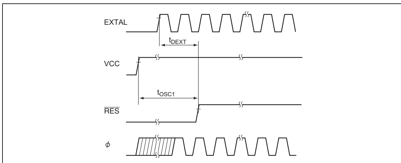
図 26.5 発振安定時間タイミング
