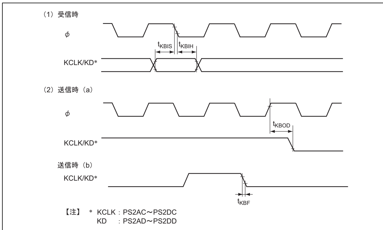
図 26.22 PS2 タイミング
