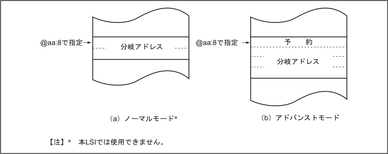
図 2.12 メモリ間接による分岐アドレスの指定
