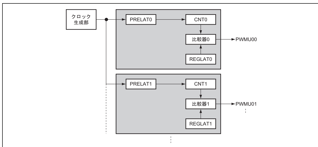
図 8.2 8 ビット単パルスモードのブロック図
