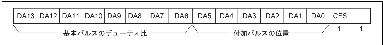
図 9.6 CFS = 1 のときの D/A データレジスタの構成
