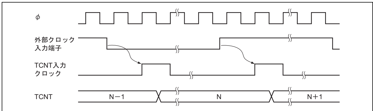
図 13.5 外部クロック動作時のカウントタイミング (両エッジの場合)
