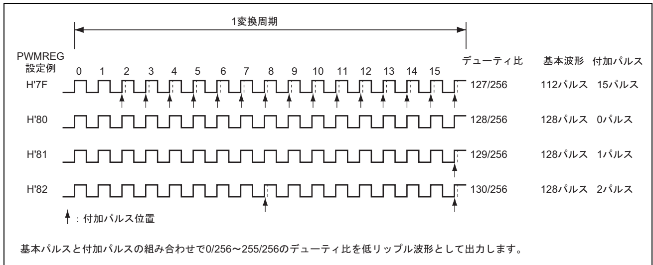
図 8.9 PWMU の設定例
