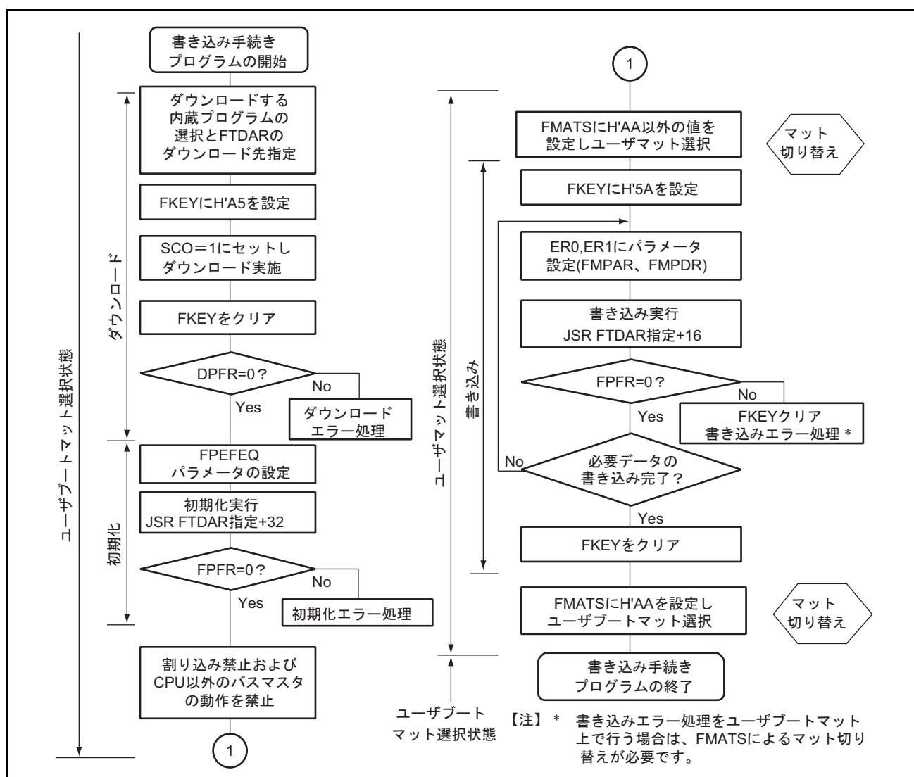
図 22.14 ユーザブートモードでのユーザマットへの書き込み手順
