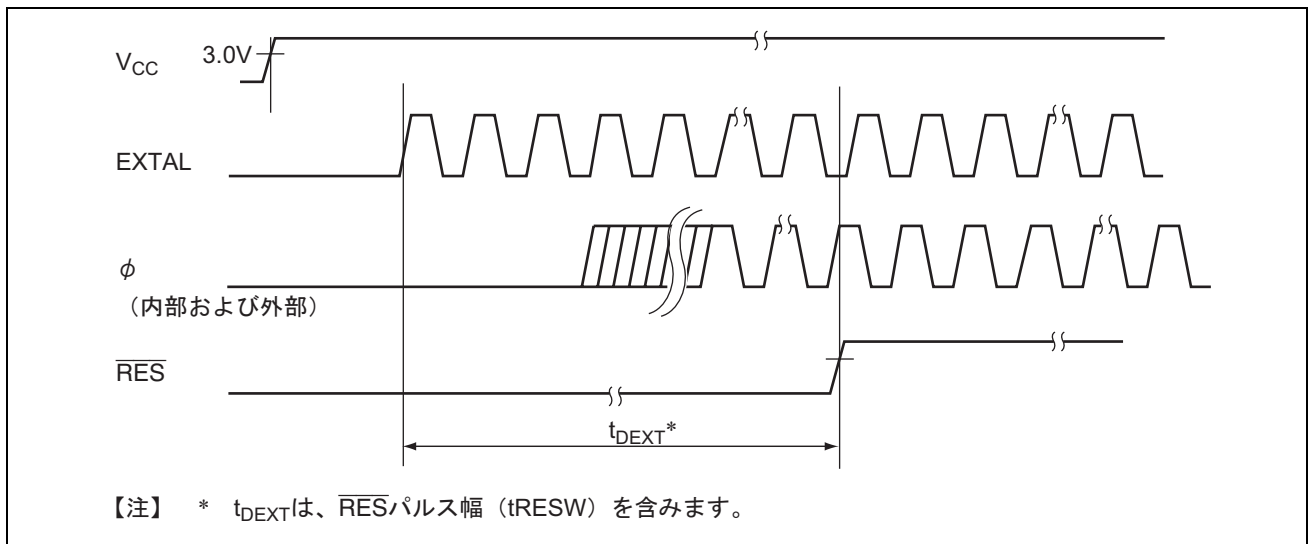
図 23.6 外部クロック出力安定遅延時間タイミング
