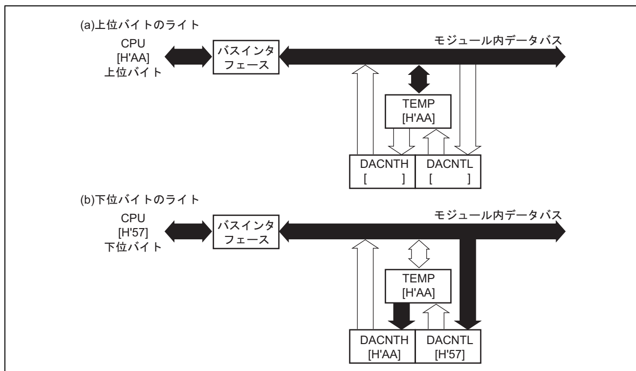
図 9.2 DACNT のアクセス動作 (1) (CPU→DACNT[H'AA57]ライト時)
