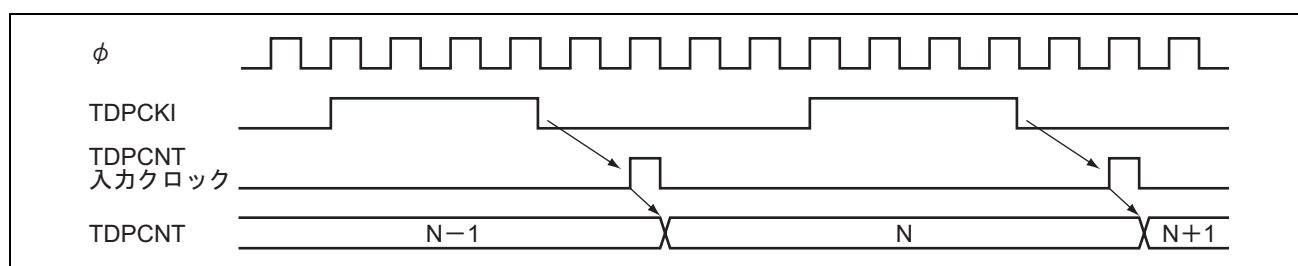
図 12.3 外部クロック動作時のカウントタイミング (立ち下がリエッジの場合)
