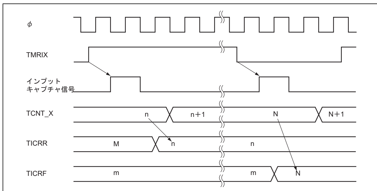
図 13.11 インพุットキャプチャ動作タイミング
