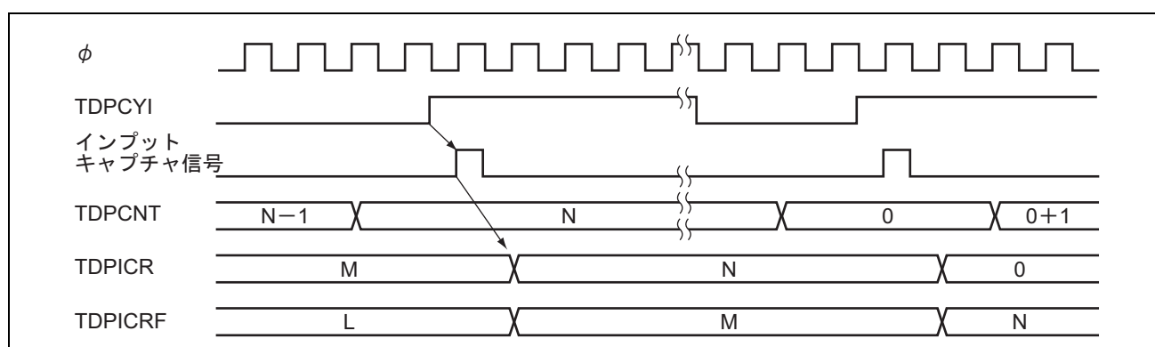
図 12.5 インพุットキャプチャのバッファ動作例
