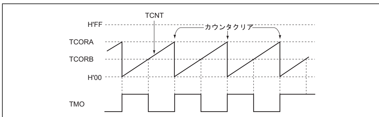
図 13.3 パルス出力例
