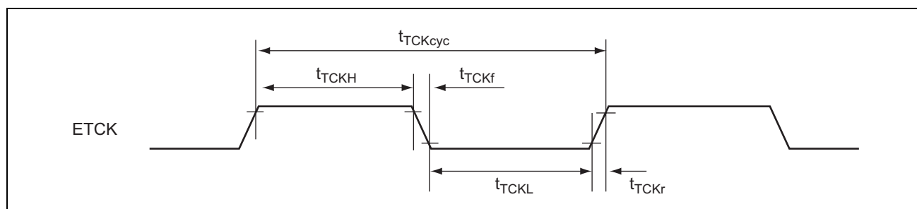
図 26.26 JTAG ETCK タイミング
