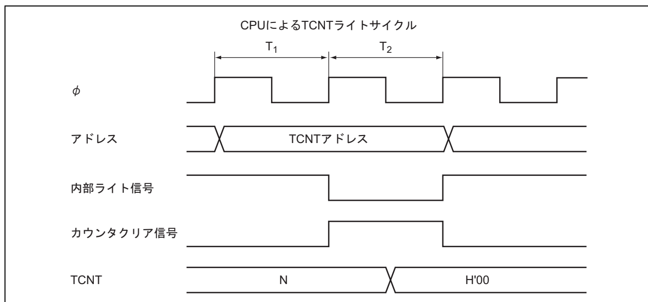
図 13.13 TCNT のライトとクリアの競合
