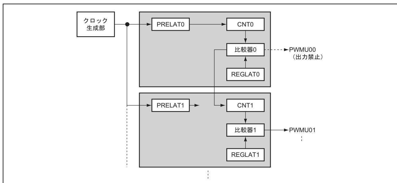
図 8.3 16 ビット単パルスモードのブロック図
