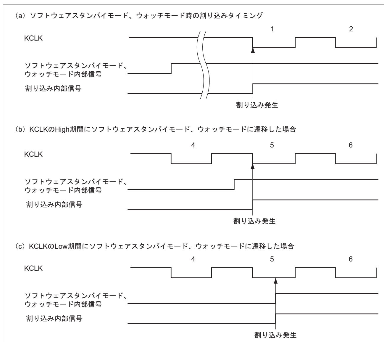
図 18.17 ソフトウェアスタンバイモード、ウォッチモード時の割り込みタイミング
