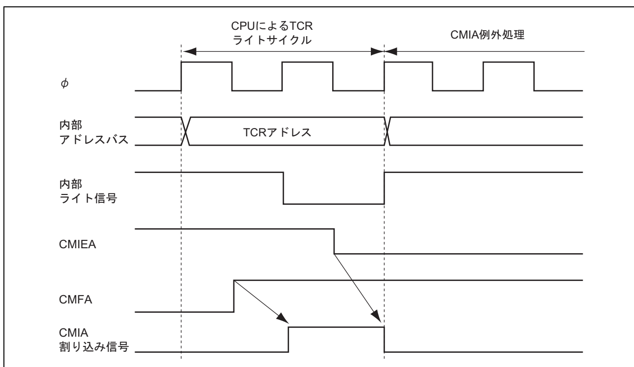
図 5.13 割り込みの発生とディスエーブルの競合
