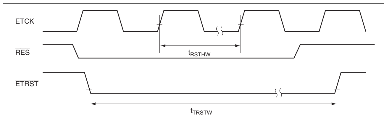
図 26.27 リセットホールドタイミング
