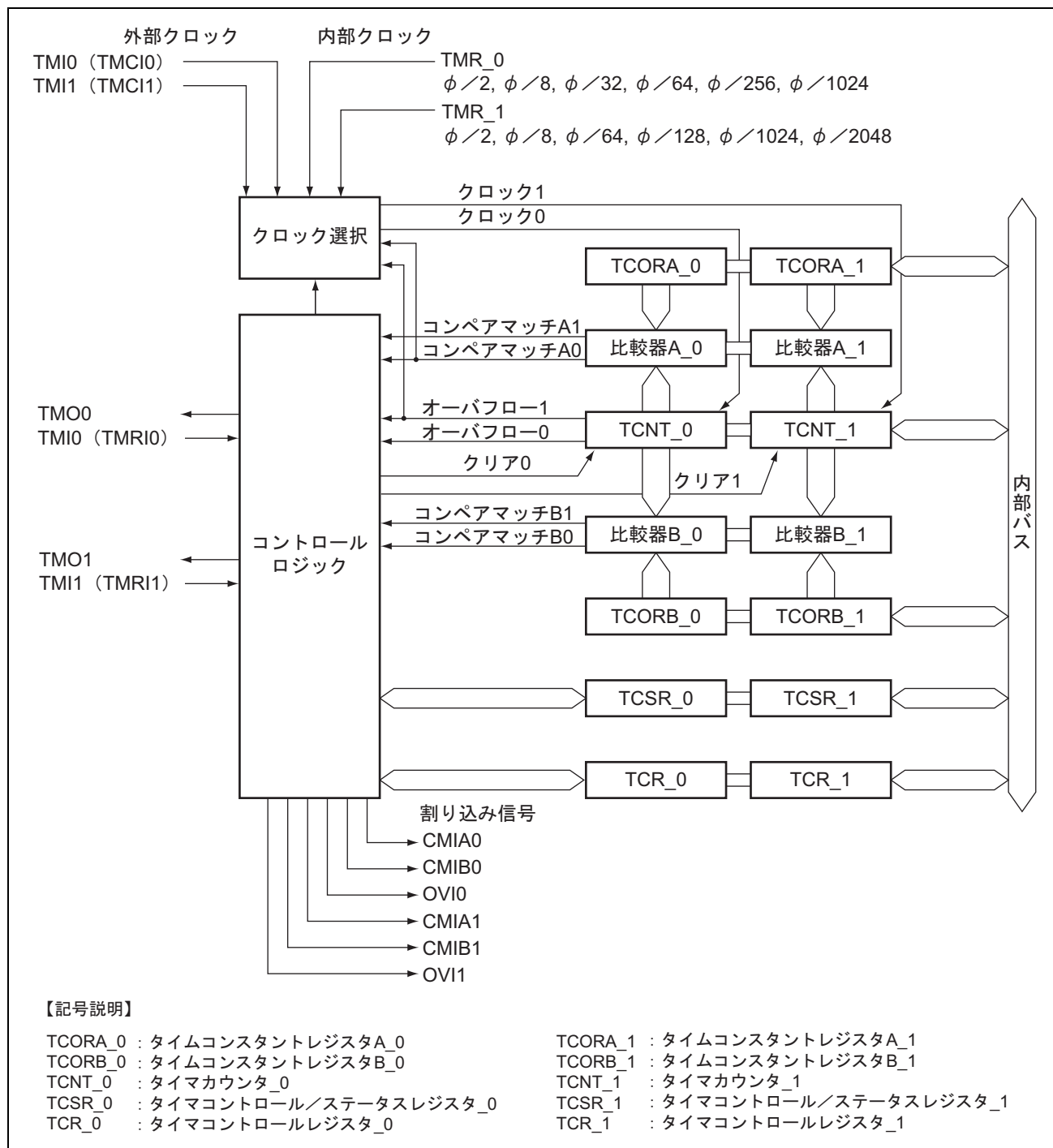
図 13.1 8 ビットタイマ (TMR_0、TMR_1) のブロック図
