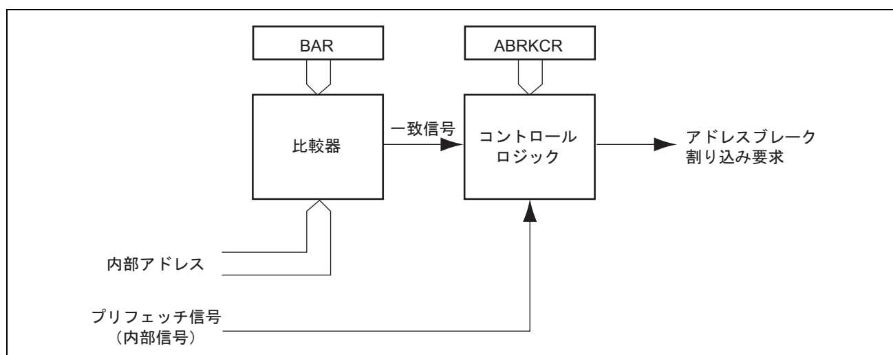
図 5.11 アドレスブレークのブロック図
