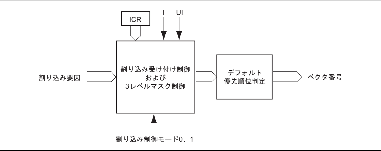
図 5.6 割り込み制御動作のブロック図
