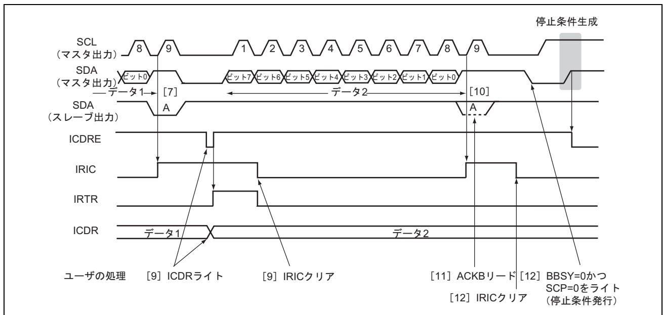
図 17.9 マスタ送信モード停止条件発行動作タイミング例 (MLS = WAIT = 0 のとき)
