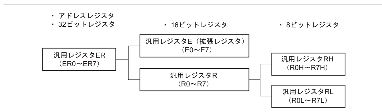
図 2.7 汎用レジスタの使用方法
