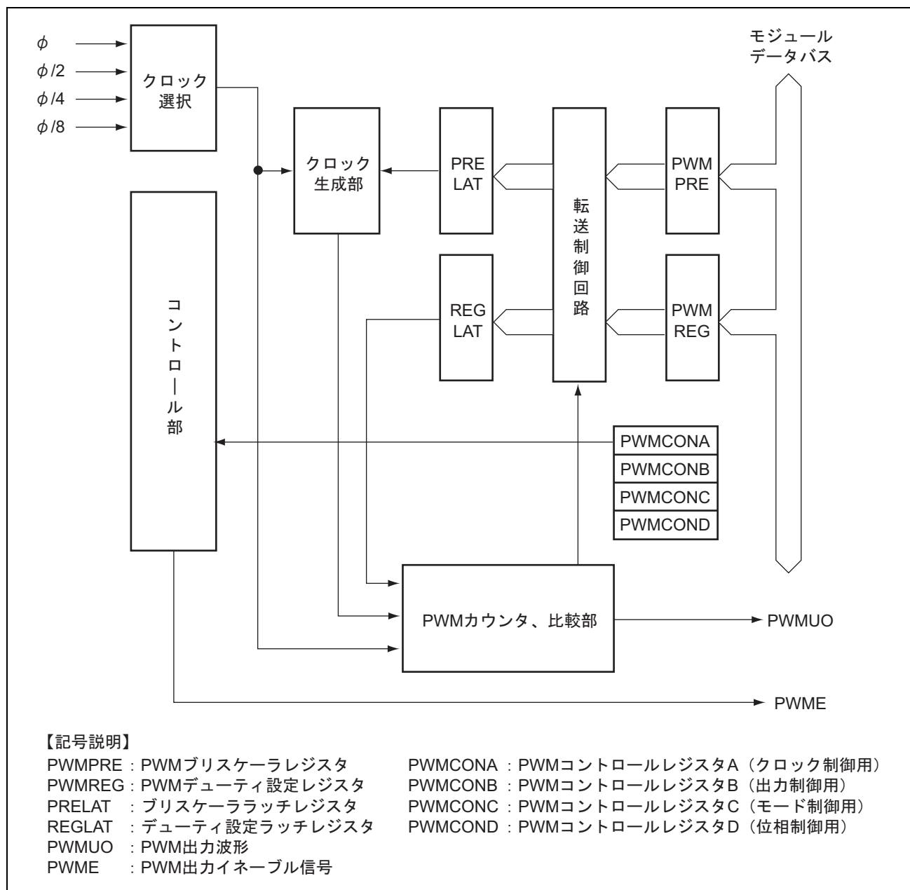
図 8.1 PWMU ブロック図
