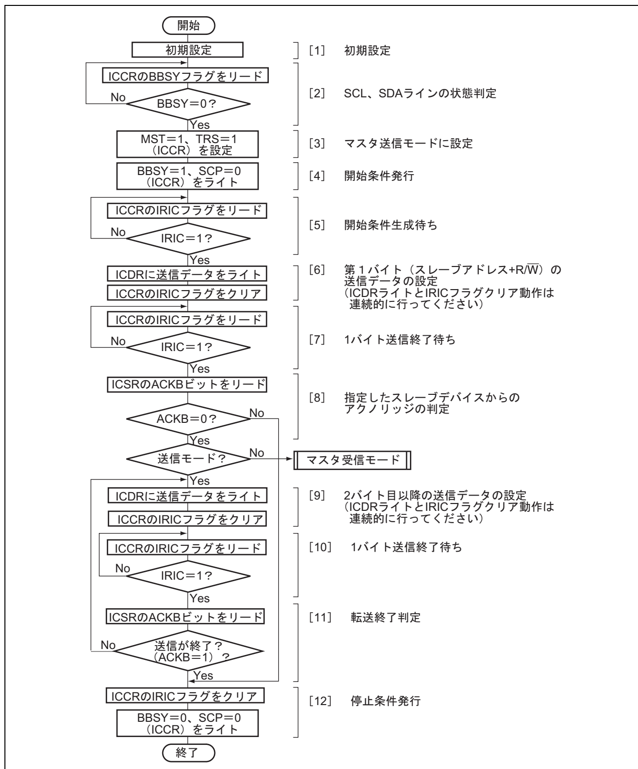
図 17.7 マスタ送信モードフローチャート例
