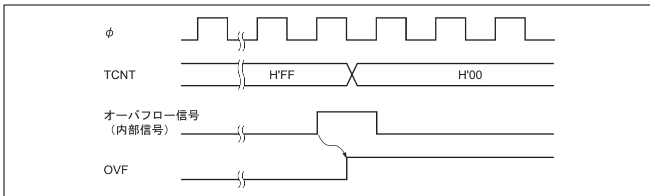
図 14.4 OVF のセットタイミング
