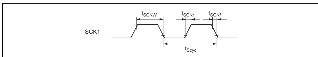
図 26.20 SCK クロック入力タイミング
