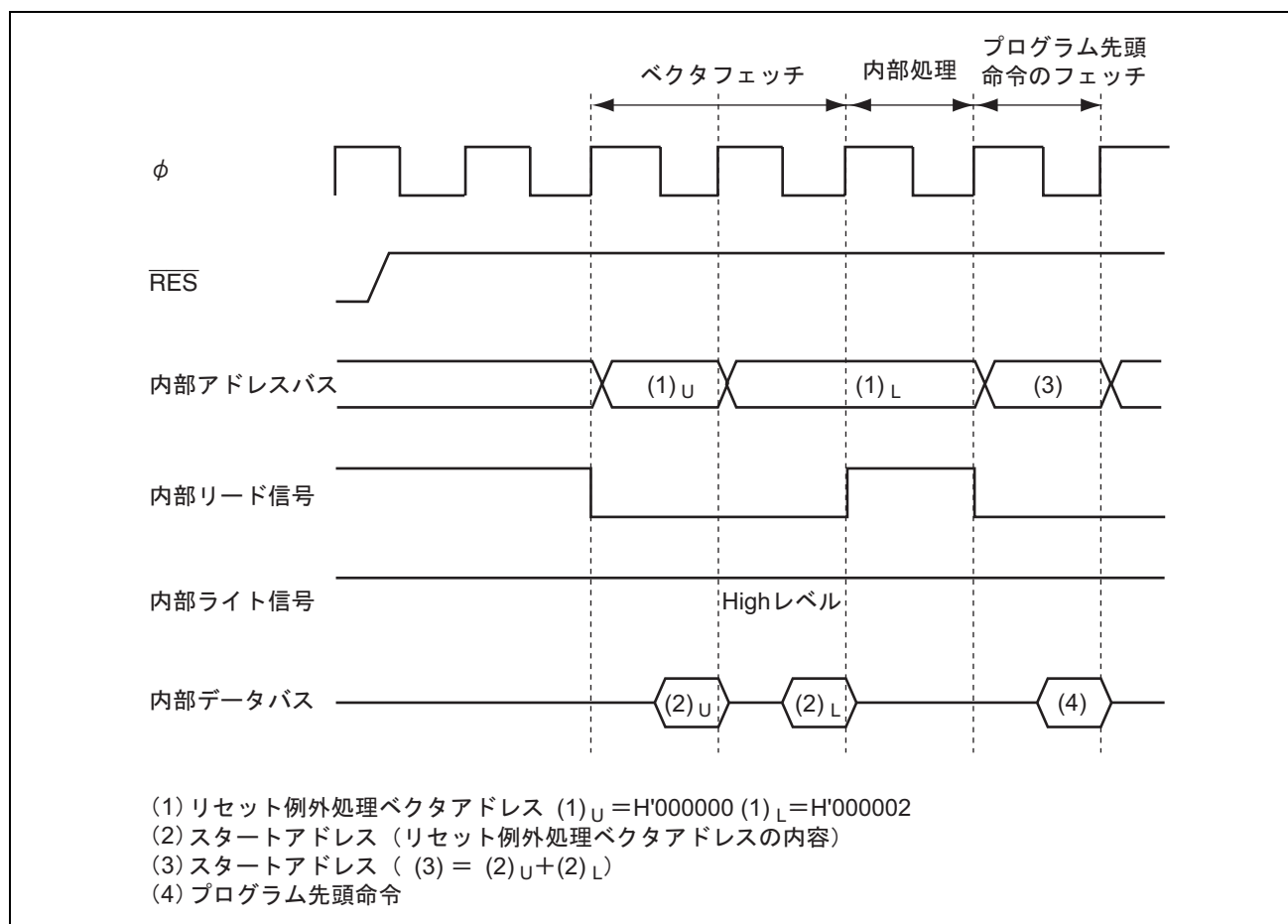
図 4.1 リセットシーケンス (モード 2)
