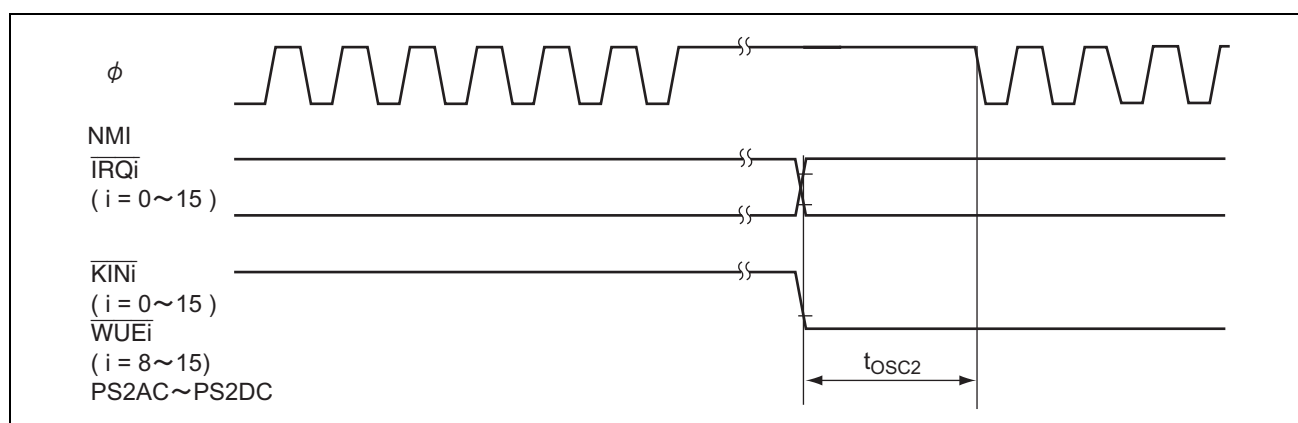
図 26.6 発振安定時間タイミング (ソフトウェアスタンバイからの復帰)
