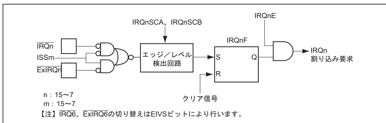
図 5.4 IRQ15 ~ IRQ7 割り込みのブロック図
