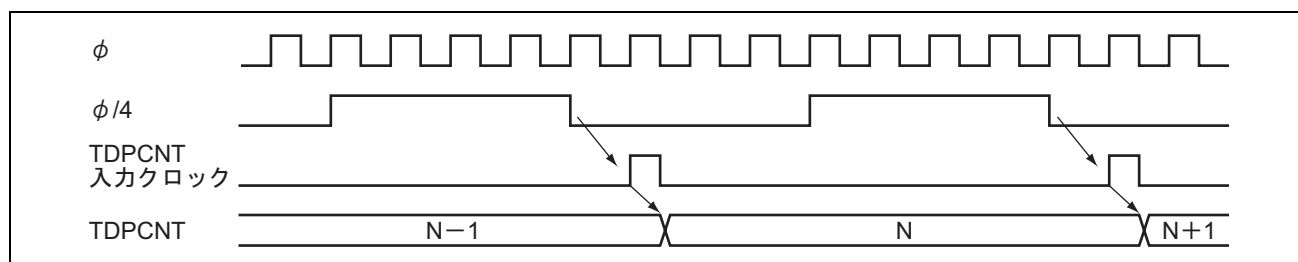
図 12.2 フリーランニングカウンタの動作例
