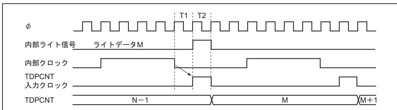
図 12.13 TDPCNT ライトとカウントアップの競合
