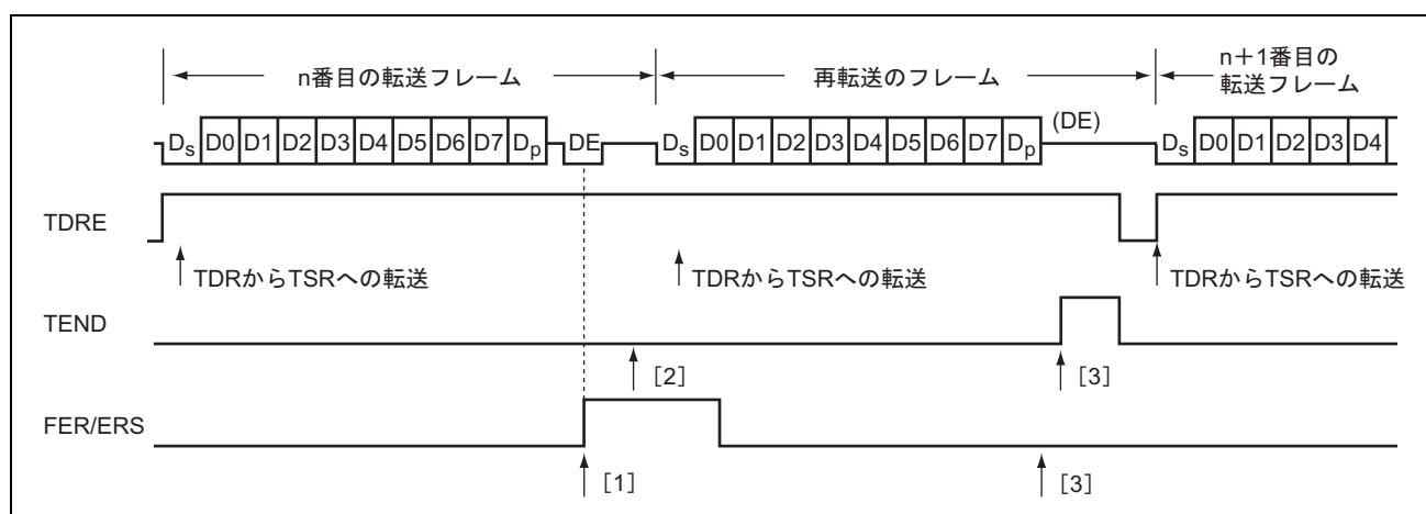
図 15.26 SCI 送信モードの場合の再転送動作
