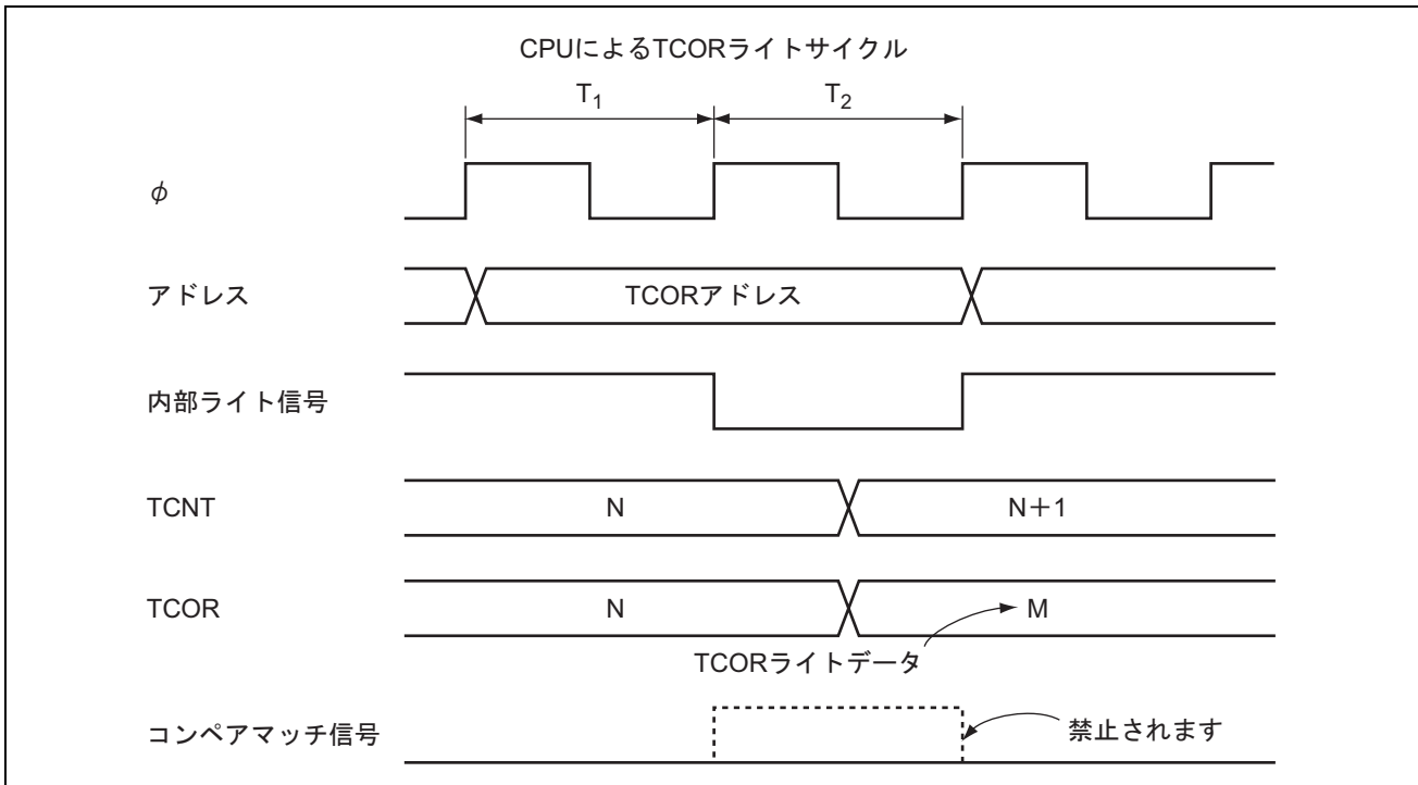
図 13.15 TCOR のライトとコンペアマッチの競合
