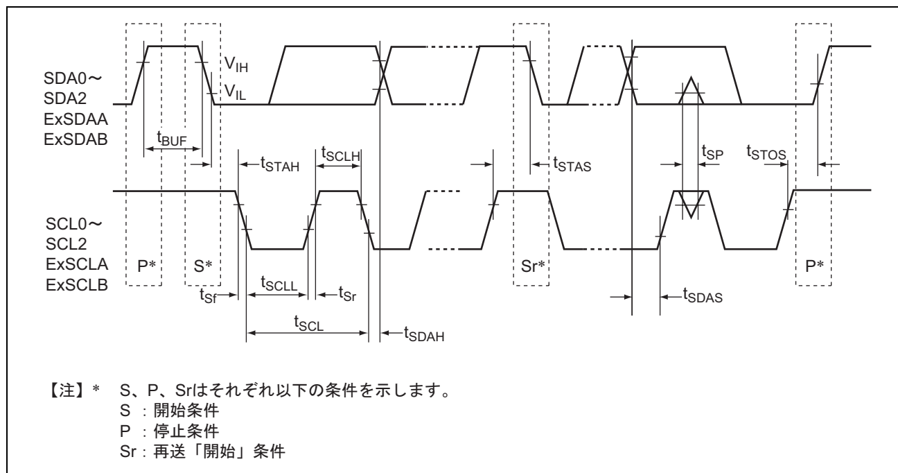
図 26.23 I 2 C バスインタフェース入出力タイミング
