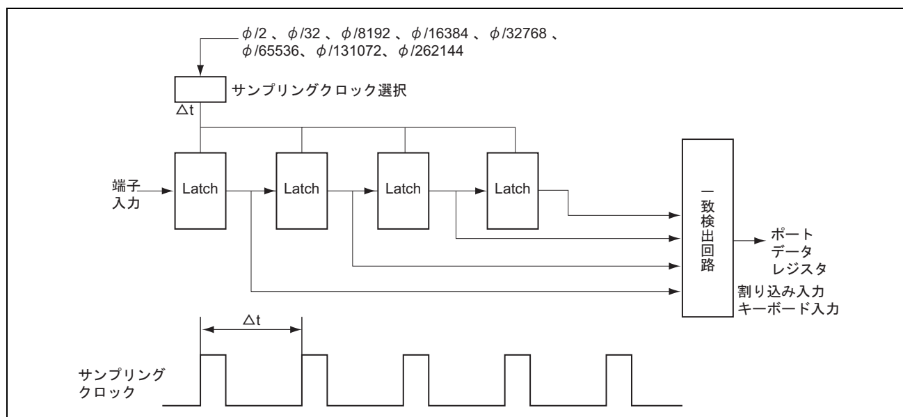
図 7.1 ノイズキャンセル回路
