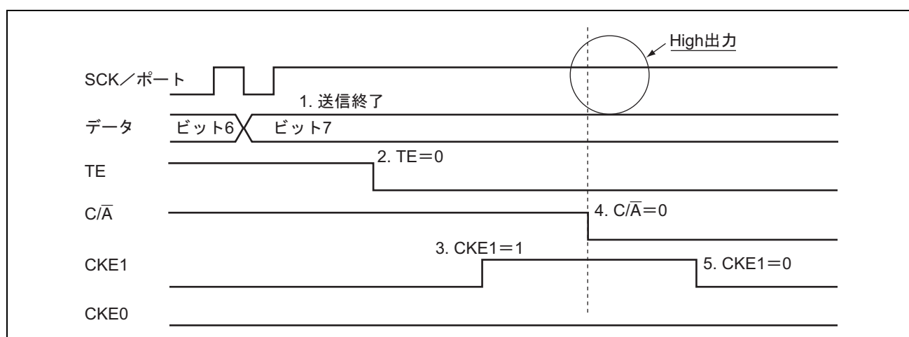
図 15.38 SCK 端子からポート端子へ切り替え時の Low 出力の回避例
