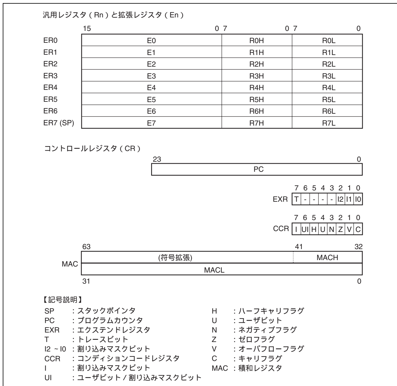
図 2.6 CPU 内部レジスタ構成
