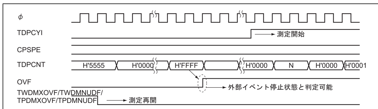
図 12.11 外部イベント停止状態のタイミング例 (2)
