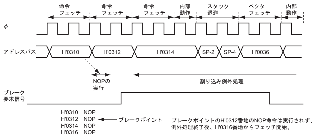
図 5.12 アドレスブレークタイミング例
