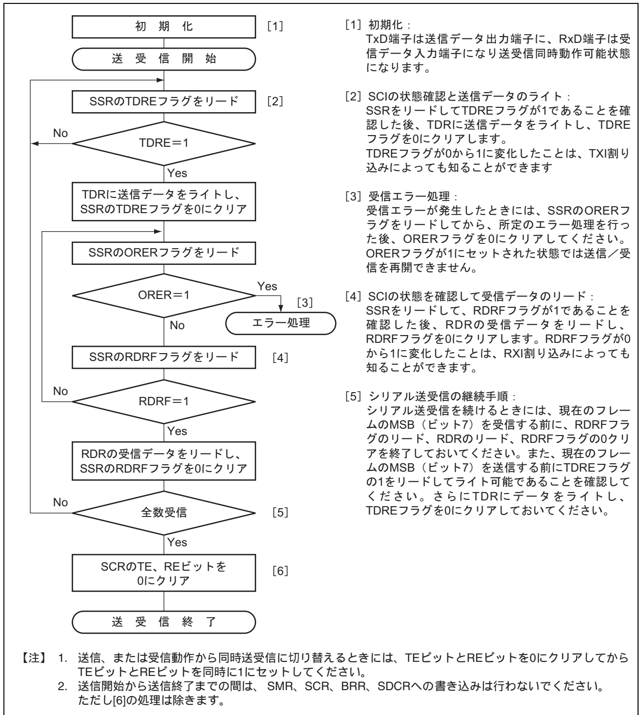
図 15.20 シリアル送受信同時動作のフローチャートの例
