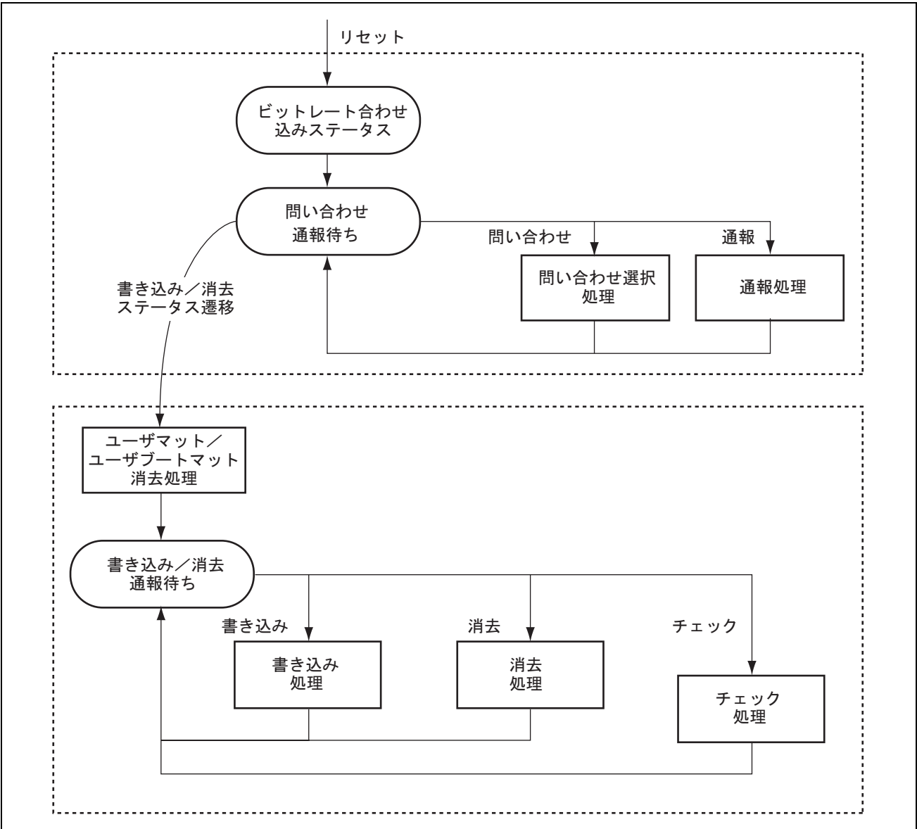
図 22.18 ブートプログラムのステータス
