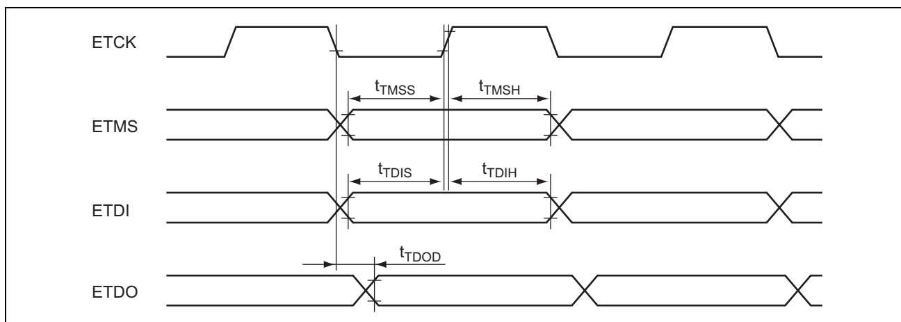
図 26.28 JTAG 入出力タイミング
