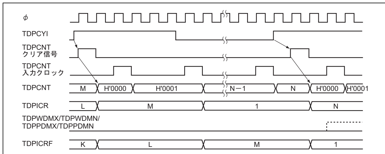
図 12.8 周期測定のタイミング例
