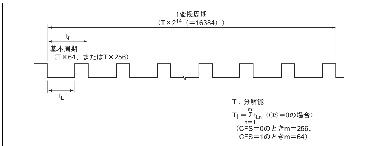
図 9.3 PWMX (D/A) の動作
