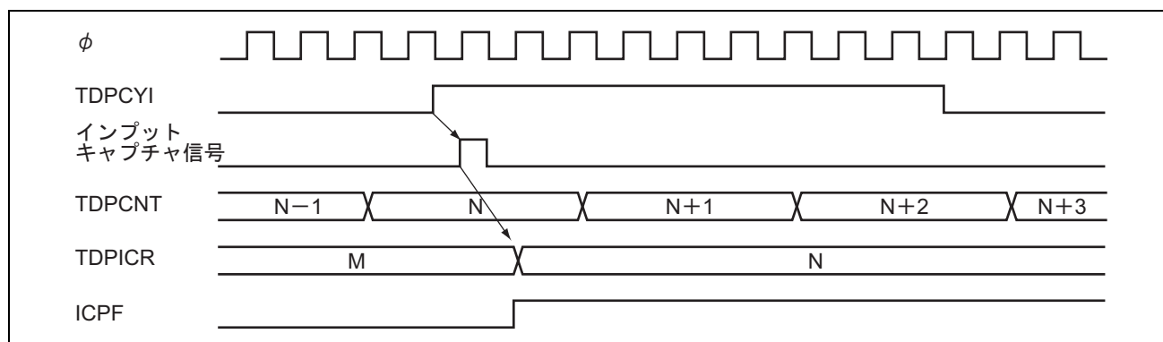
図 12.4 インพุットキャプチャ動作タイミング例 (立ち上がりエッジ選択時)
