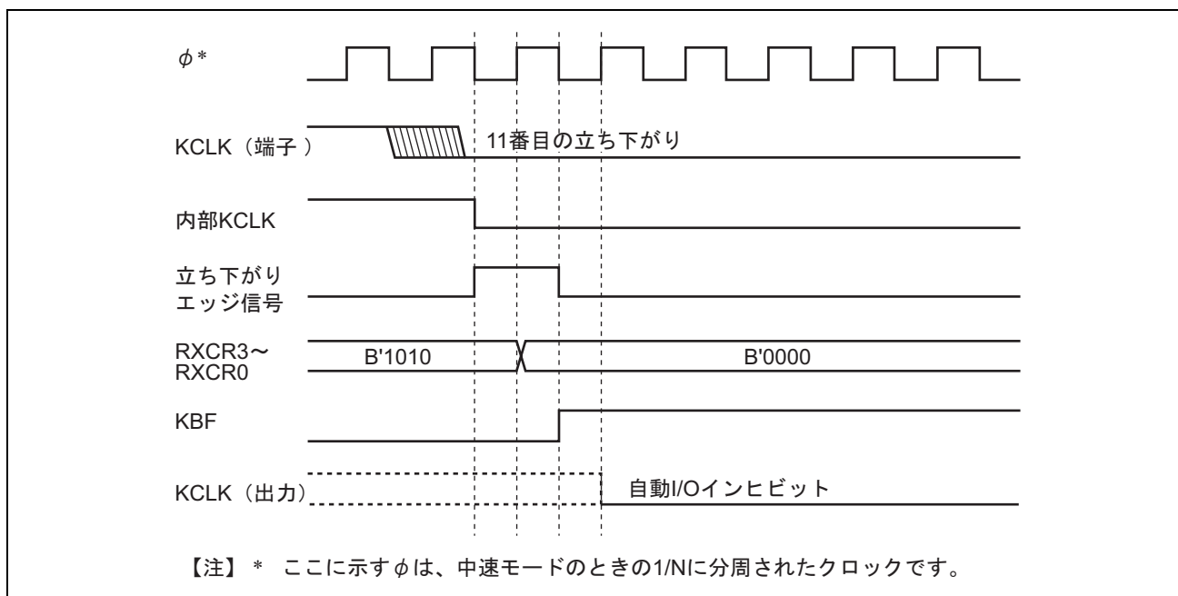
図 18.11 KBF セットと KCLK 自動 I/O インヒビット生成のタイミング
