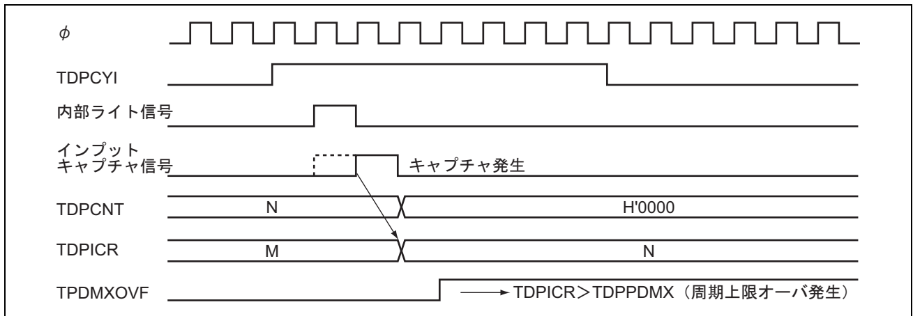
図 12.16 エッジ検出とレジスタライトの競合 (周期測定モード)
