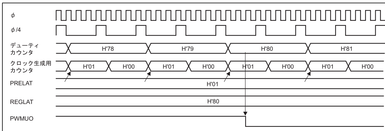
図 8.4 デューティカウンタとクロック生成用カウンタの動作例 ( カウントクロックソースに \phi/4 を選択、PWMPRE = H'01、PWMREG = H'80 に設定した場合 )
