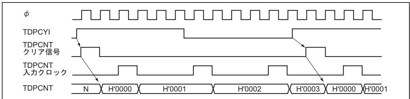
図 12.7 周期測定モード時のカウンタの動作例
