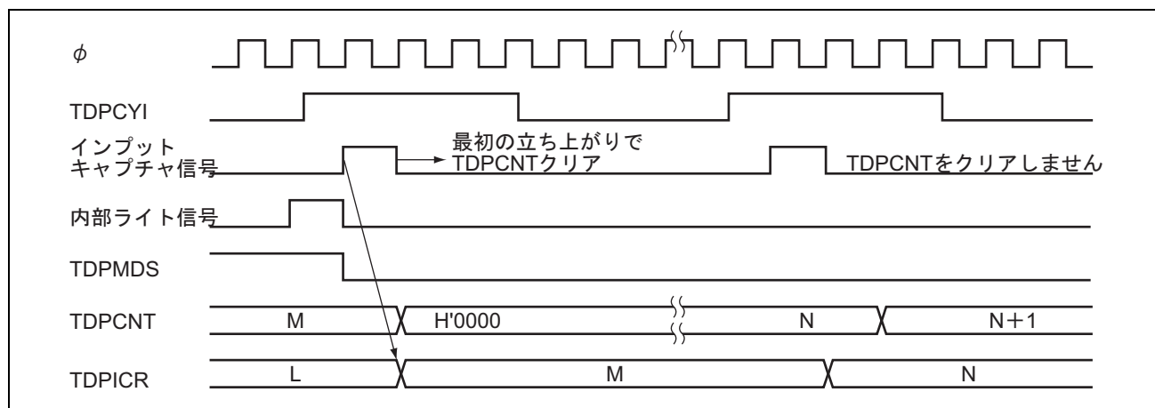
図 12.17 エッジ検出と TDPMDS クリアの競合 (周期測定モードからタイマモードへの切り替え)
