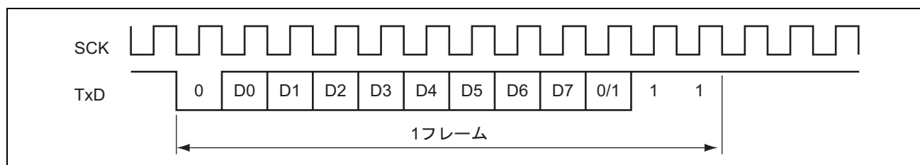
図 15.4 出力クロックと送信データの位相関係 (調歩同期式モード)
