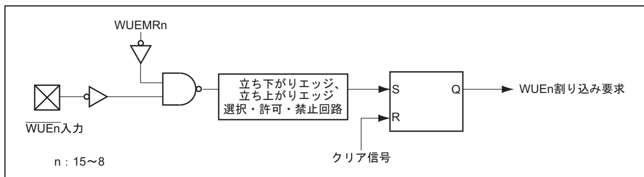
図 5.5 WUE15 ~ WUE8 割り込みのブロック図
