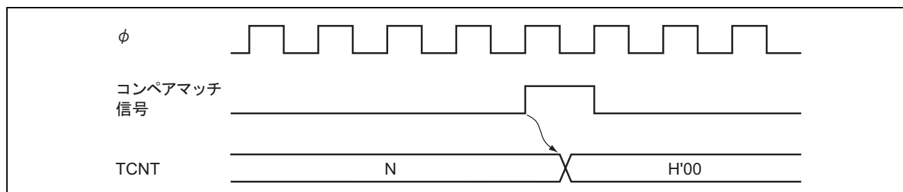
図 13.8 コンペアマッチによるカウンタクリアタイミング
