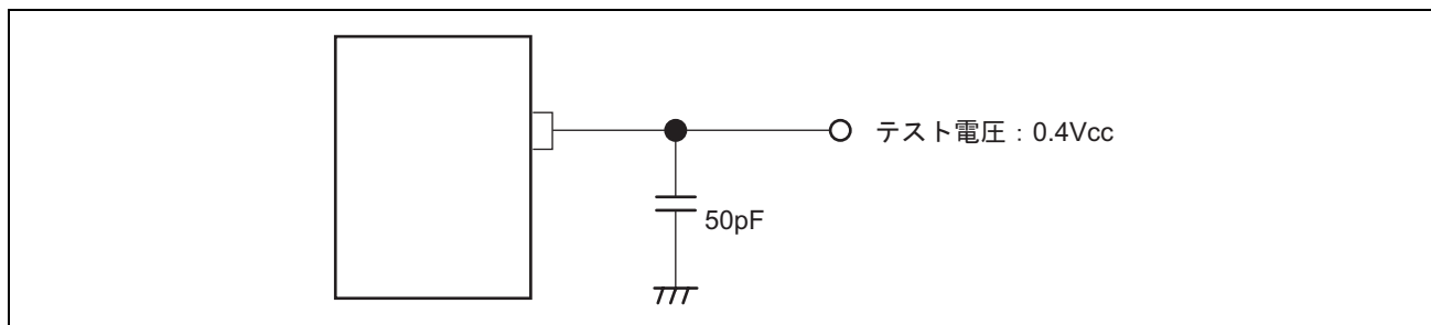
図 26.25 テスタ測定条件
