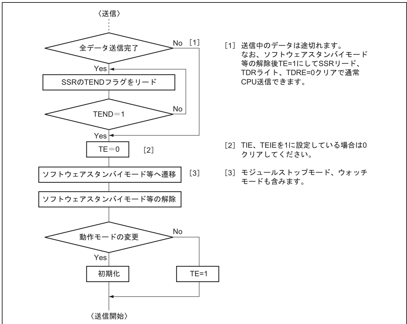
図 15.33 送信時のモード遷移フローチャートの例
