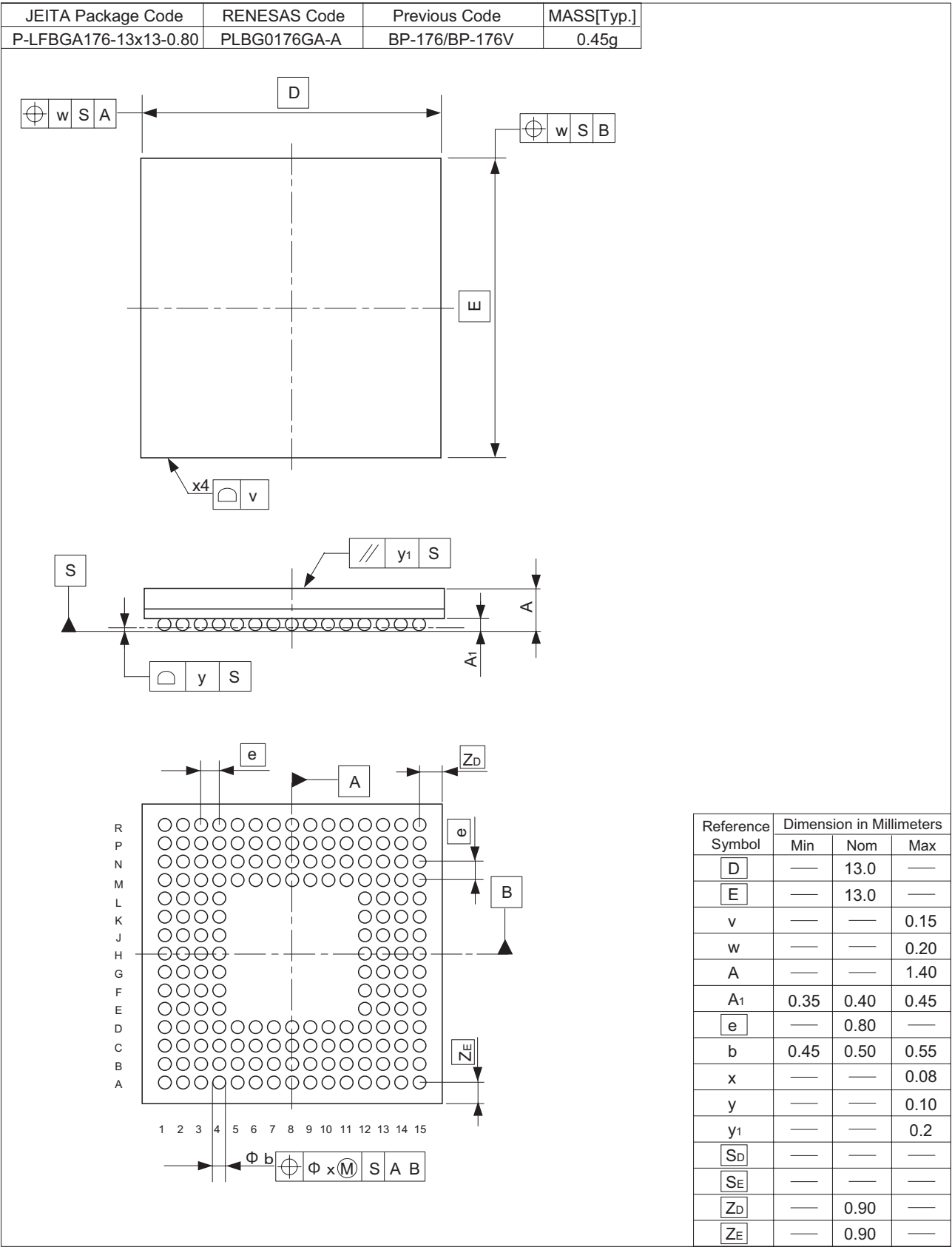
図 C.2 外形寸法図 (BP-176V)
