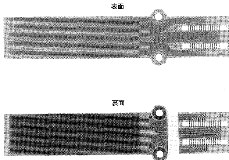
図 2-3 フレキシブル基板
