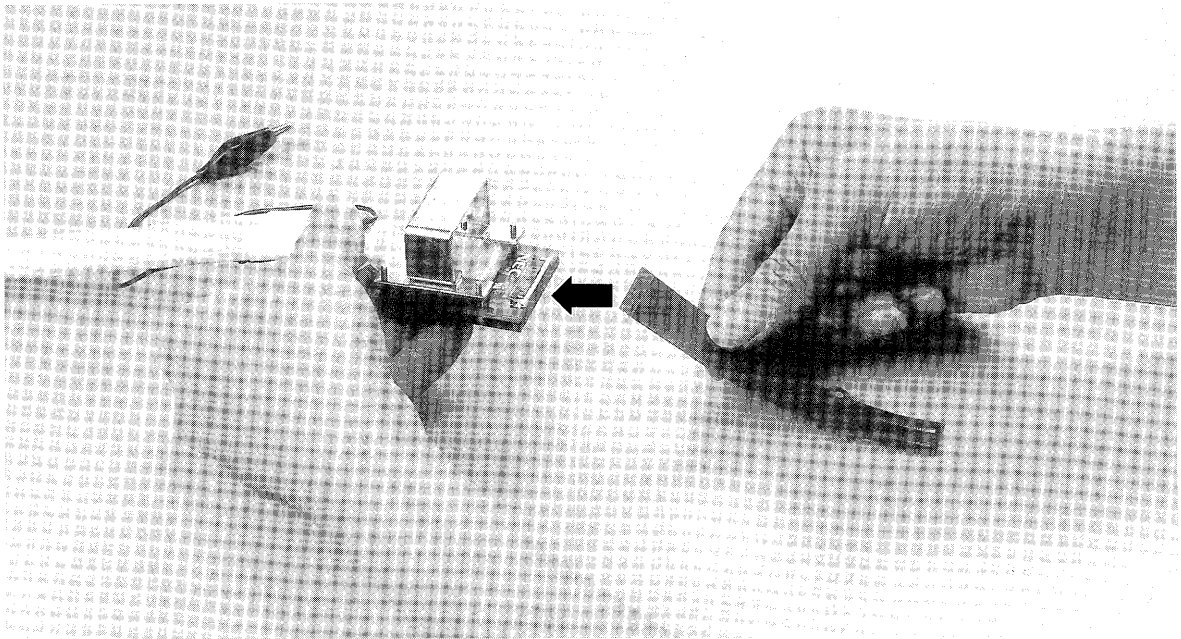
図2-4 エミュレーション・プローブの接続
