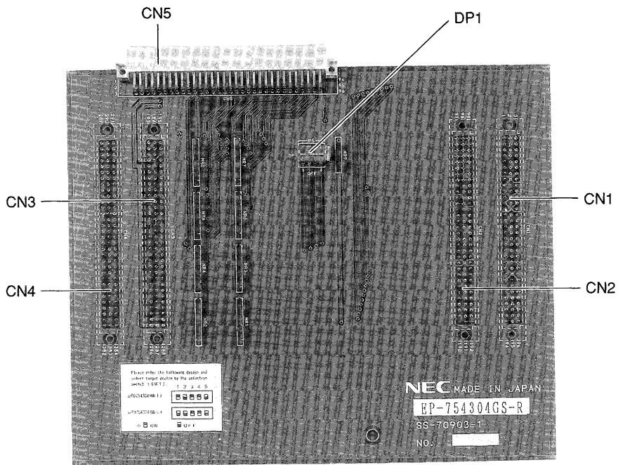
図1-3 アダプタ・ボード
