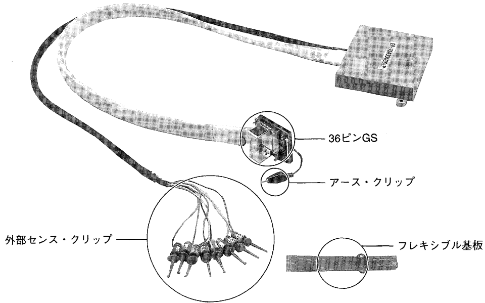
図1-3 アダプタ・ボード
