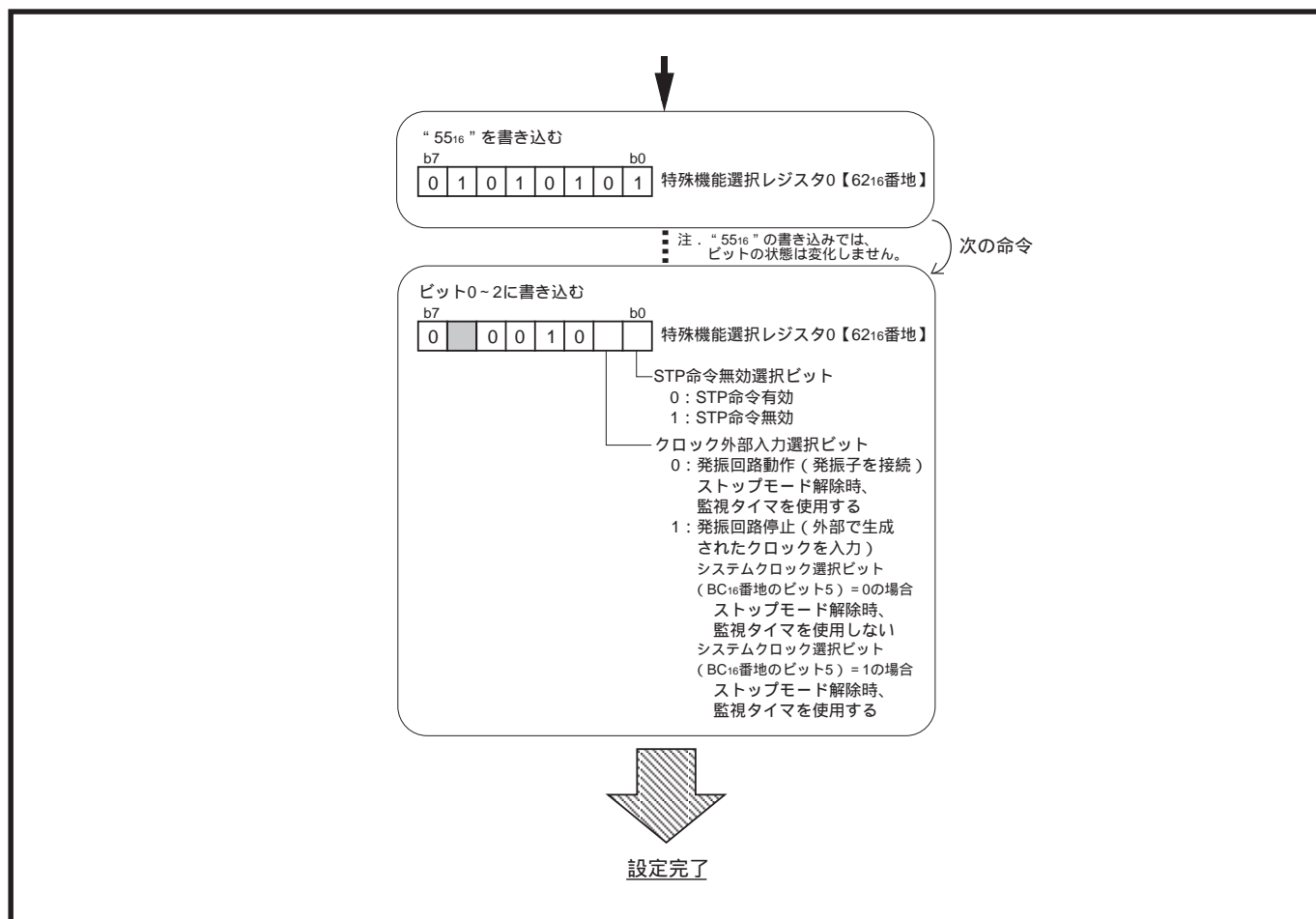
図16.2.3 特殊機能選択レジスタ0への書き込み手順
