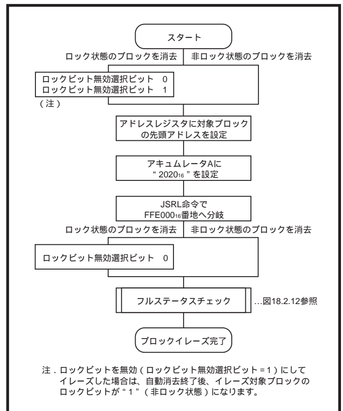
図18.2.7 ブロックイレーズフローチャート
