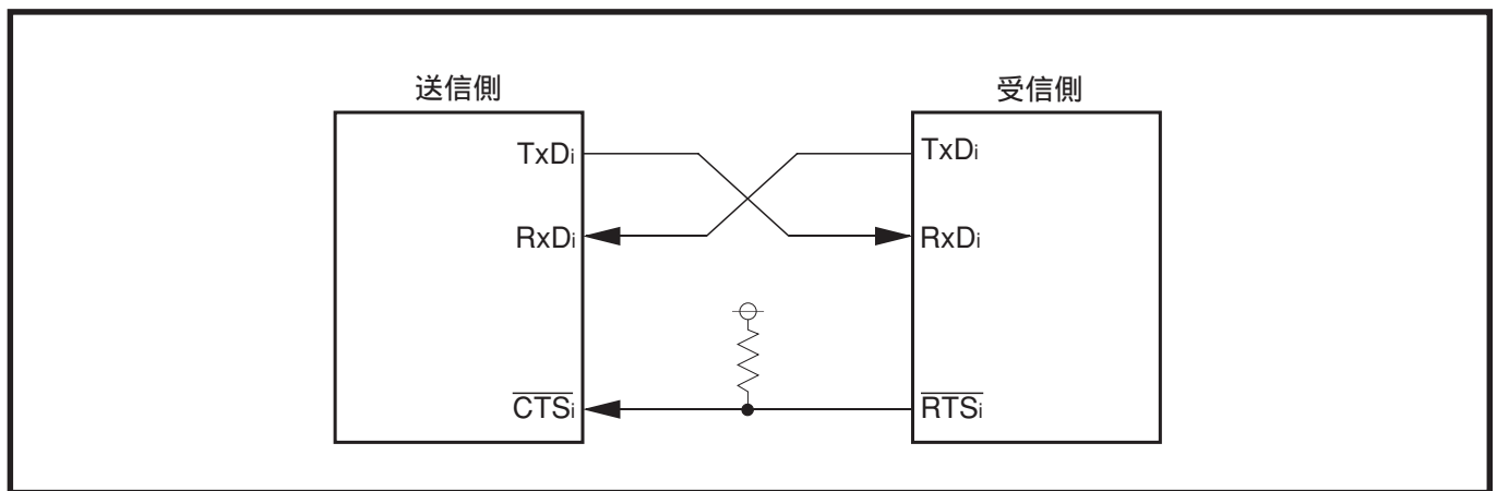
図12.4.12 結線例
