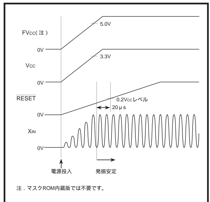
図4.1.3 パワーオンリセット条件
