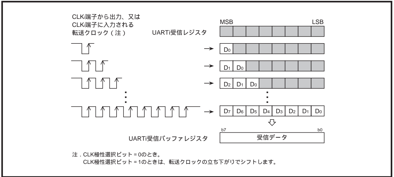
図12.3.11 受信動作
