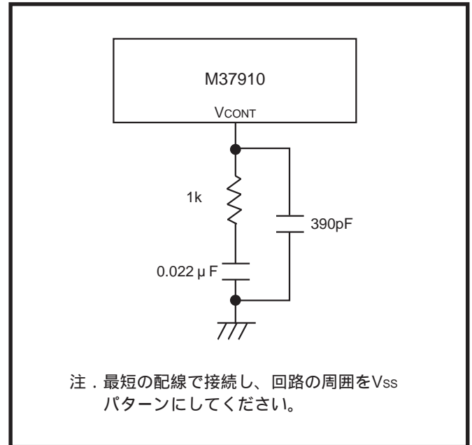
図5.1.3 フィルタ回路接続例
