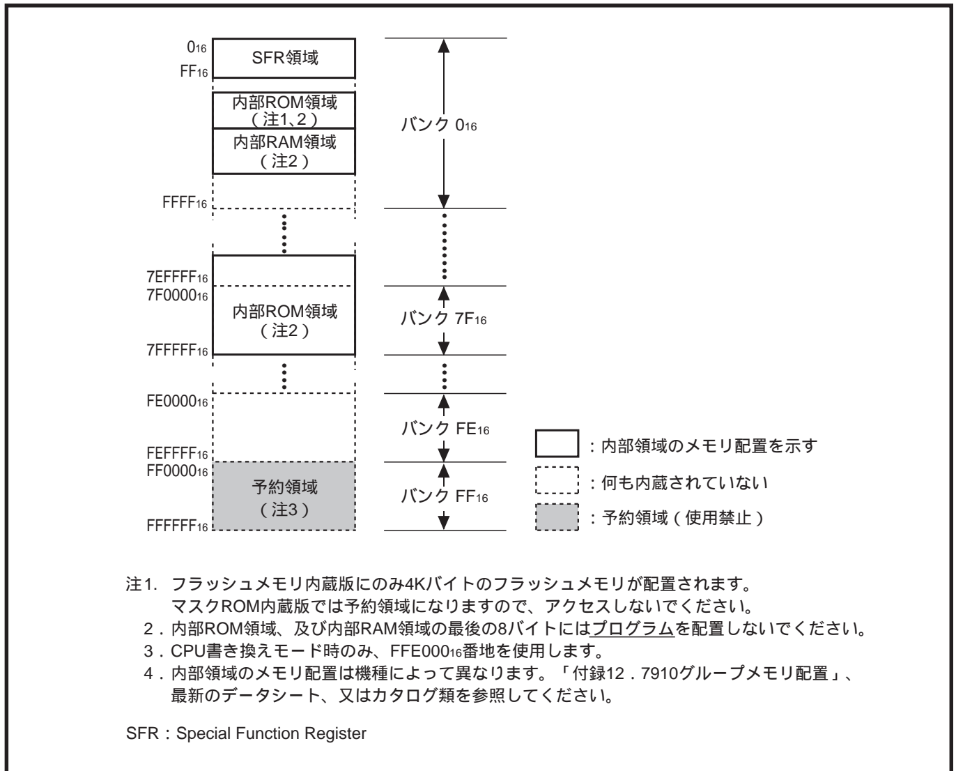
図2.3.1 M37910のアクセス空間
