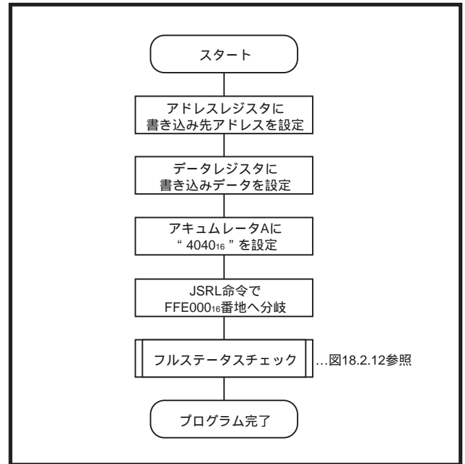
図18.2.6 プログラムフローチャート
