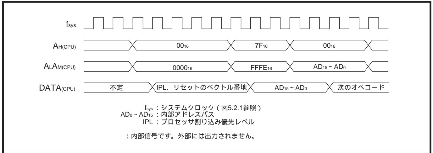
図4.4.1 リセット後の内部処理シーケンス
