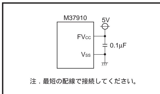
図18.1.1 FV CC - V SS 間のバイパスコンデンサ
