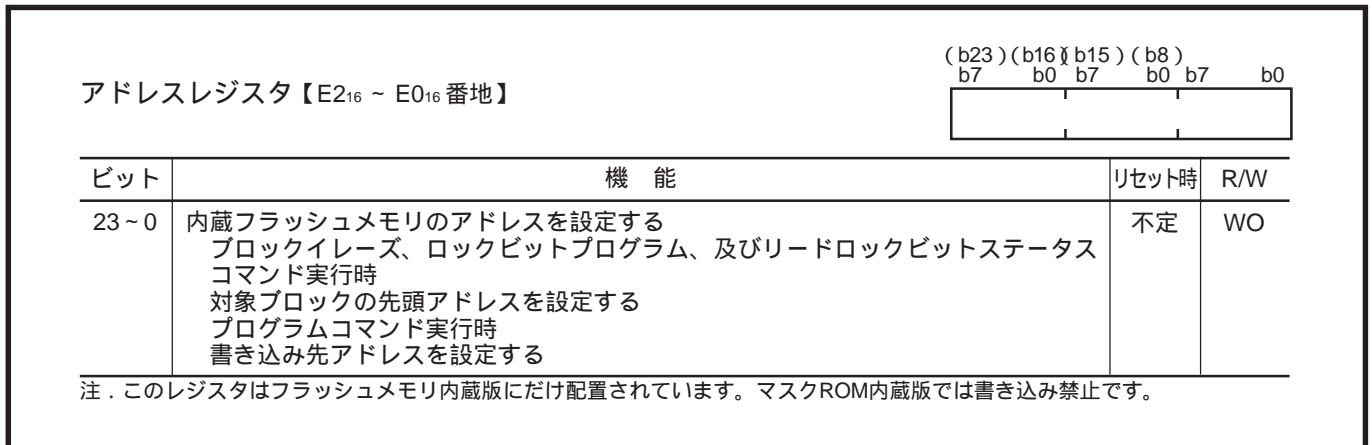
図18.2.1 アドレスレジスタのレジスタ構成
