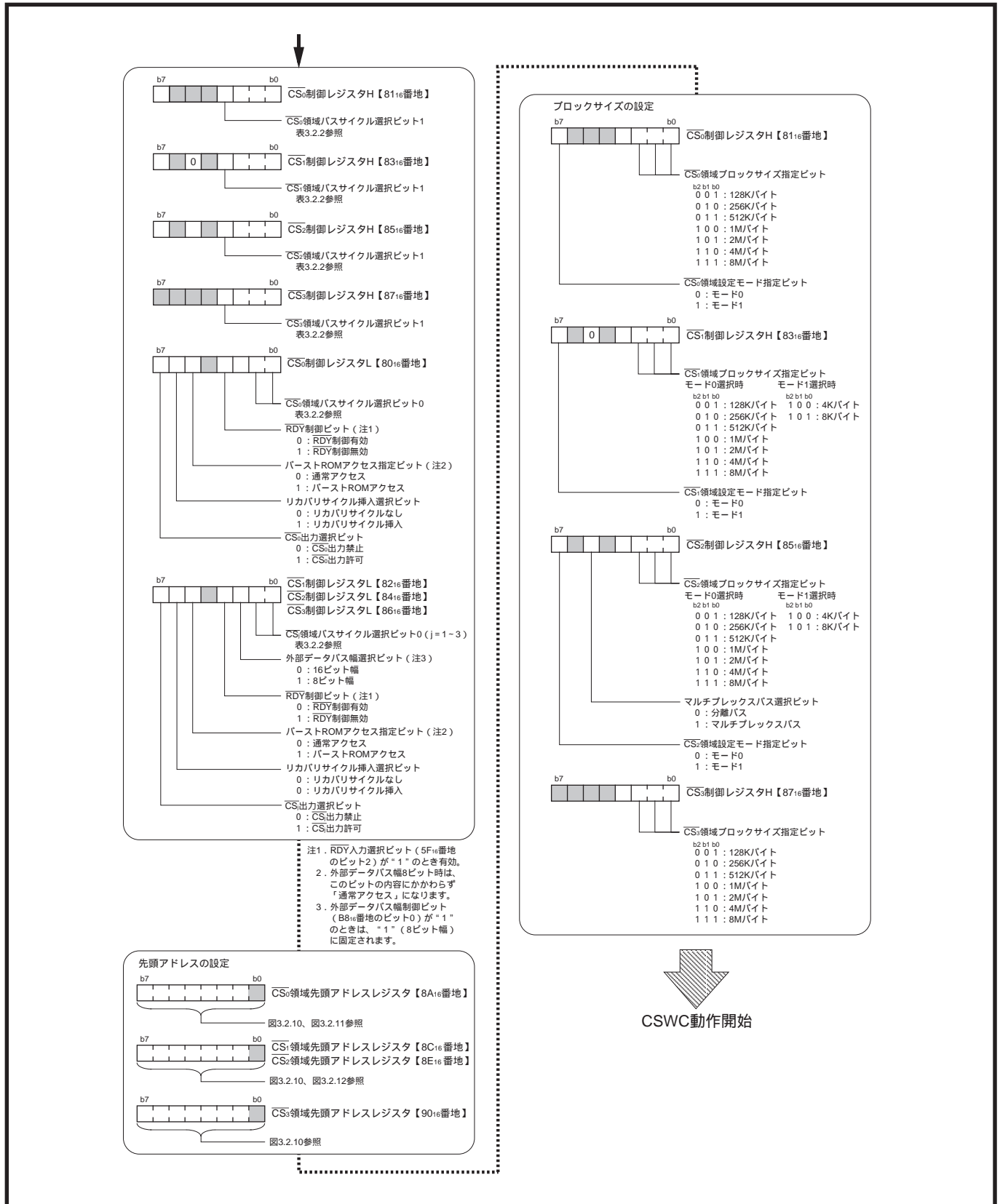
図3.2.16 CSWC関連レジスタの初期設定例
