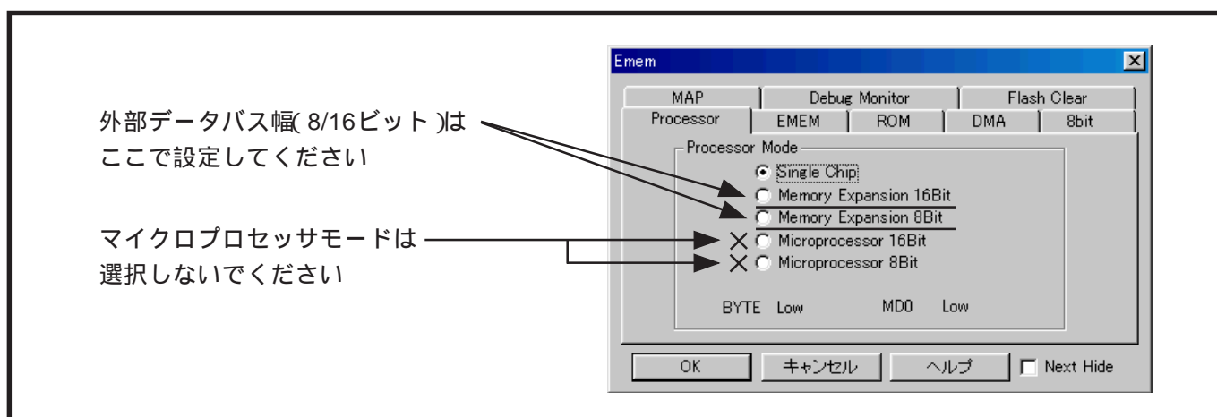
図16 外部データバス幅設定例
