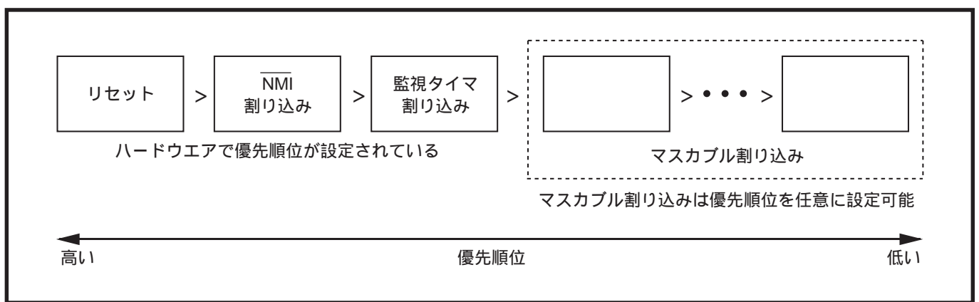
図7.4.1 ハードウェアで設定されている割り込み優先順位
