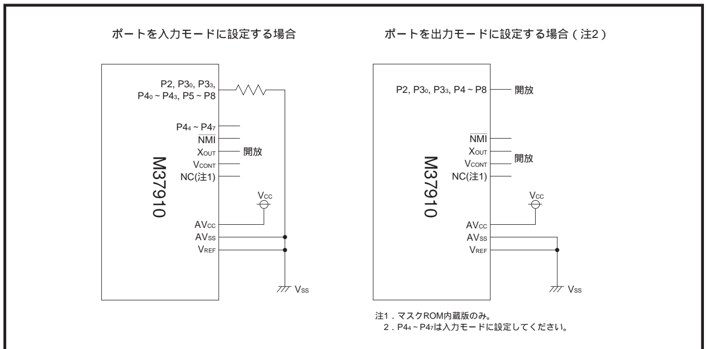
図6.3.2 メモリ拡張モード時の未使用端子の処理例
