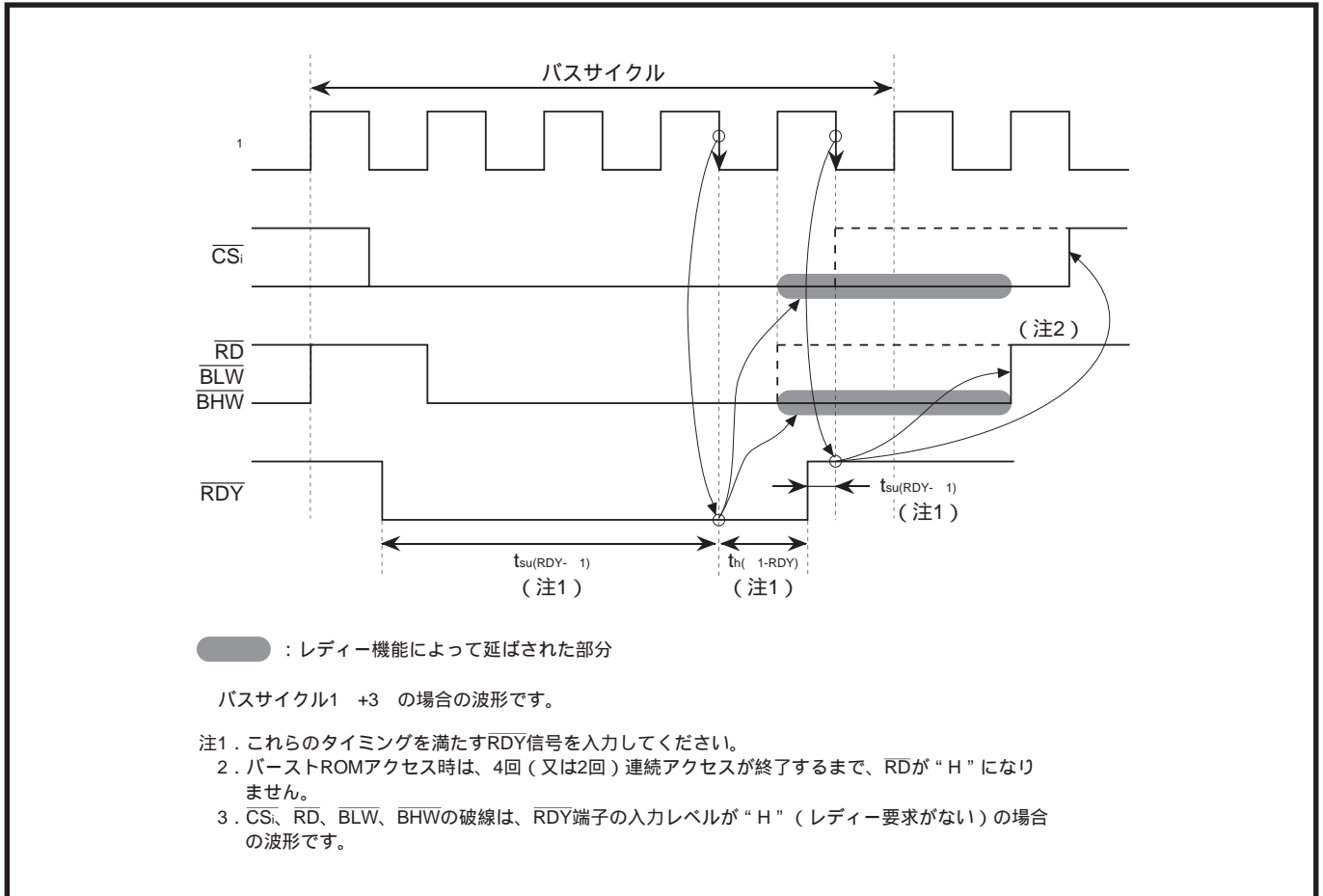
図3.3.3 レディー要求受付、及びレディー状態解除タイミング(RDY解除タイミング選択ビット=1時)
