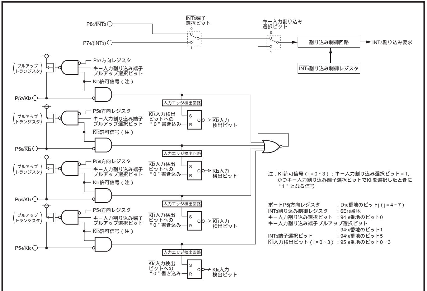
図8.2.1 キー入力割り込み機能ブロック図
