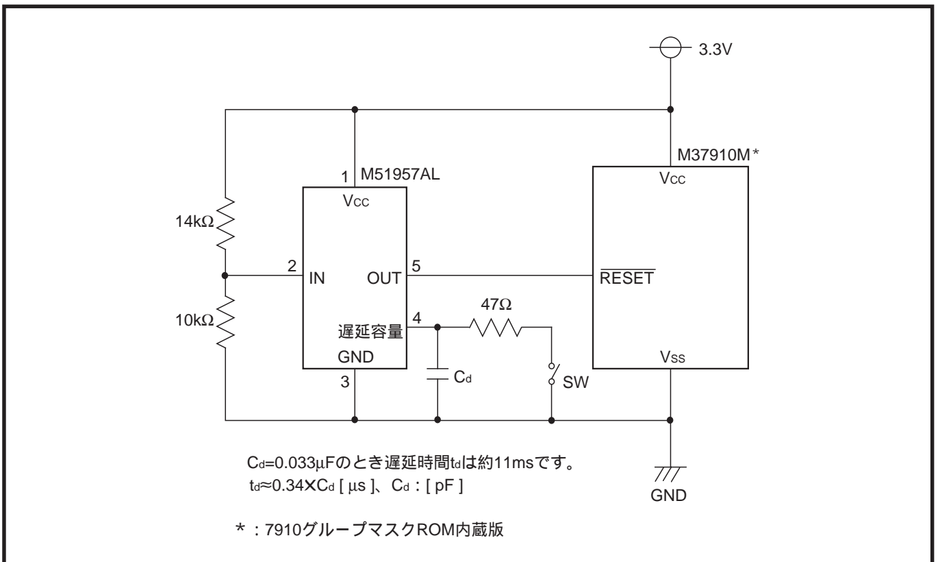
図4.1.5 パワーオンリセット回路例(2)(マスクROM内蔵版)
