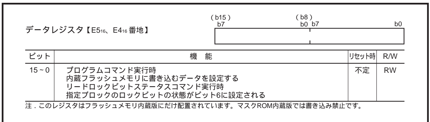
図18.2.2 データレジスタのレジスタ構成
