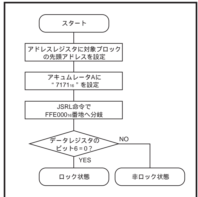
図18.2.9 リードロックビットステータスフローチャート
