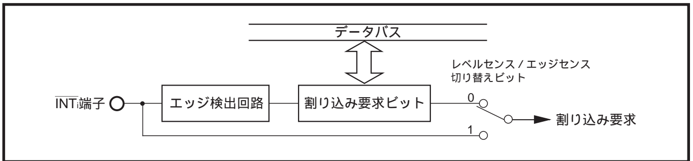
図7.10.5 INT i 割り込み要求
