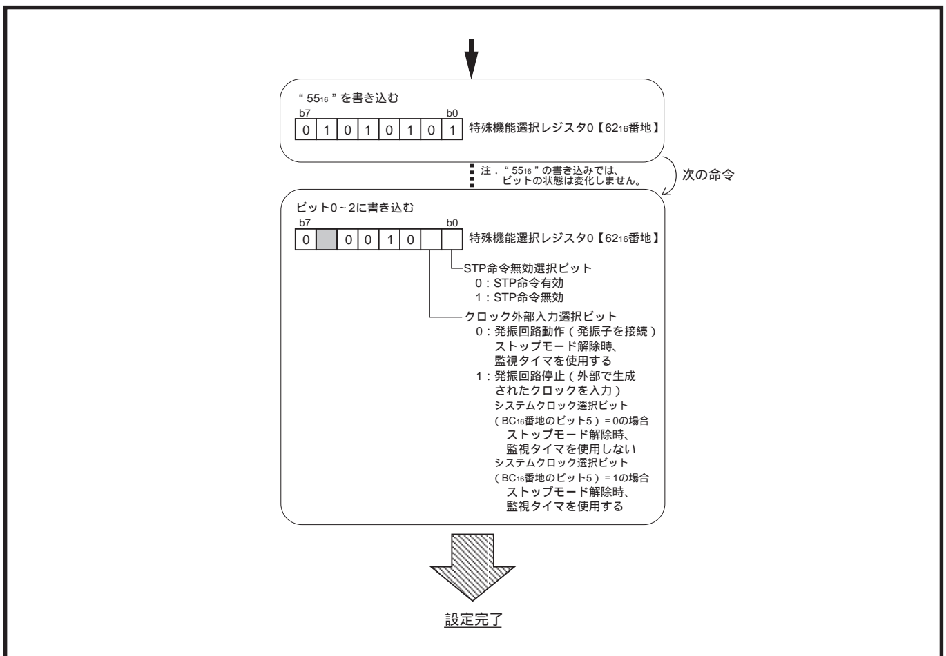
図5.2.3 特殊機能選択レジスタ0への書き込み手順
