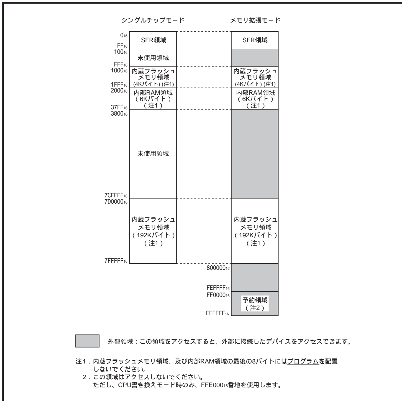
図18.1.2 M37910FEMHPの各プロセッサモード時のメモリ配置
