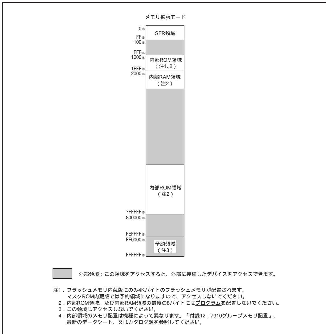
図3.1.2 M37910の外部領域
