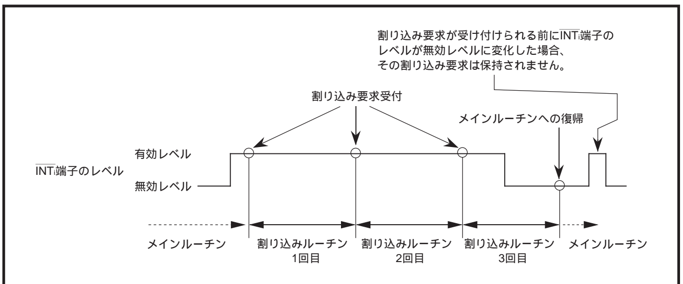
図7.10.6 INT i 割り込み要求(レベルセンス選択時)
