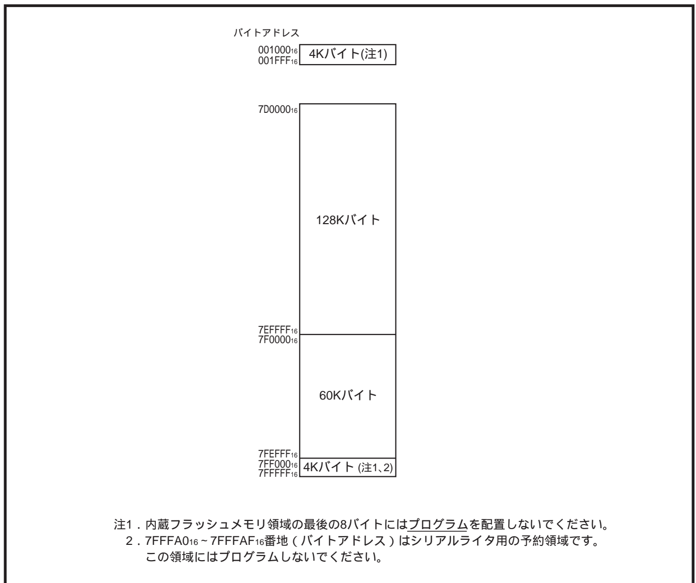
図18.1.3 M37910FEMHPの内蔵フラッシュメモリのメモリ配置
