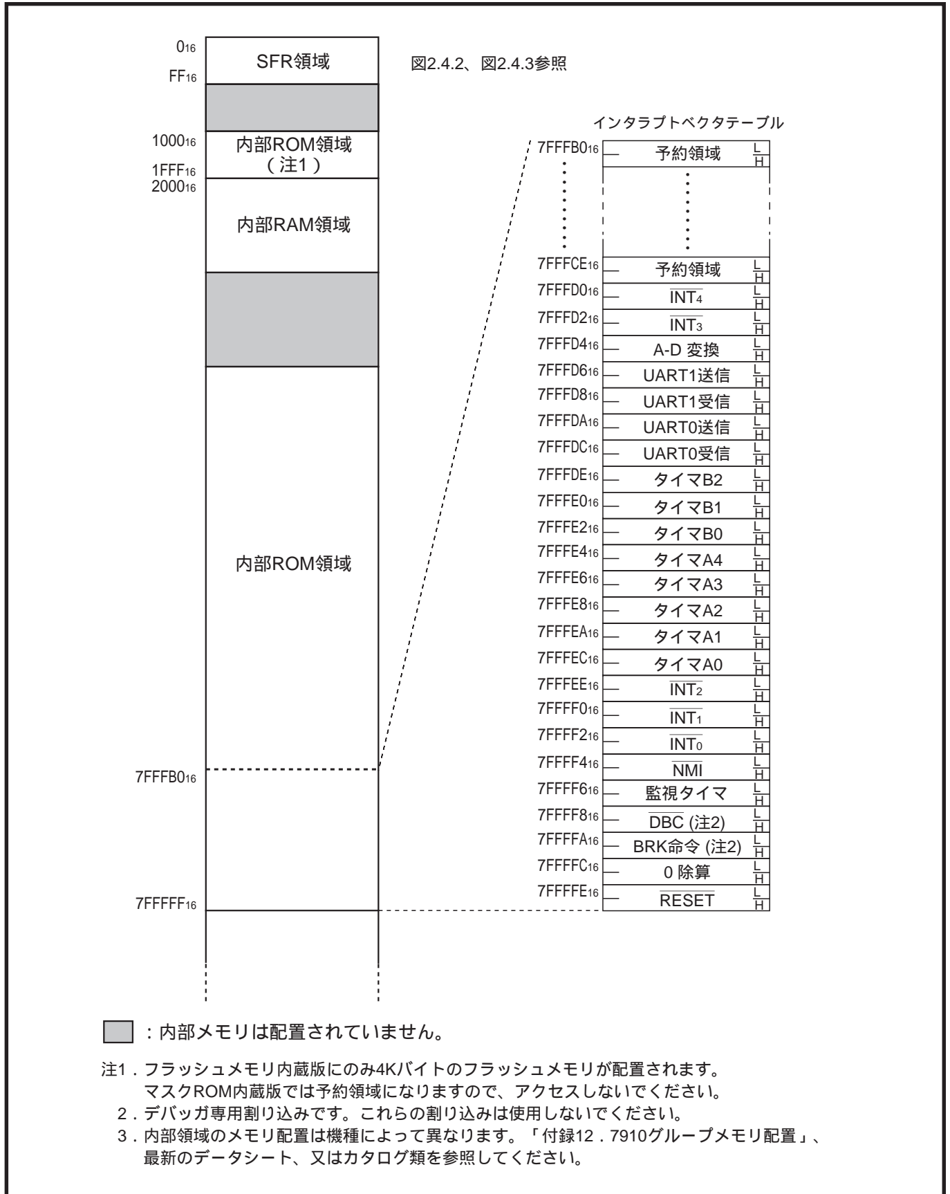
図2.4.1 M37910の内部領域のメモリ配置図
