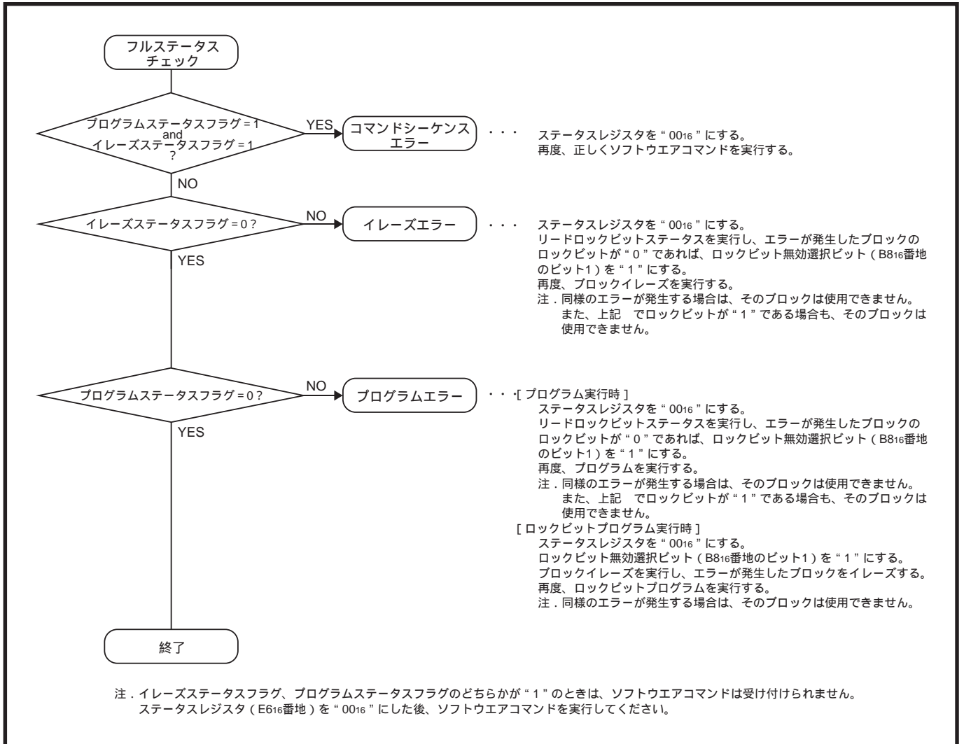
図18.2.12 フルステータスチェックフローチャート及び各エラー発生時の対処方法
