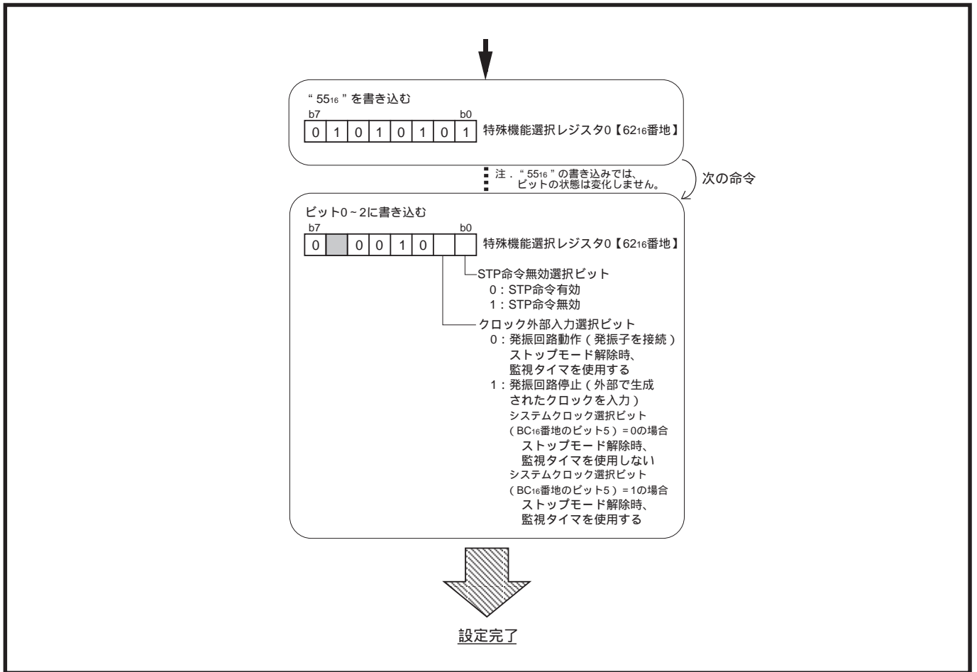
図17.1.2 特殊機能選択レジスタ0への書き込み手順
