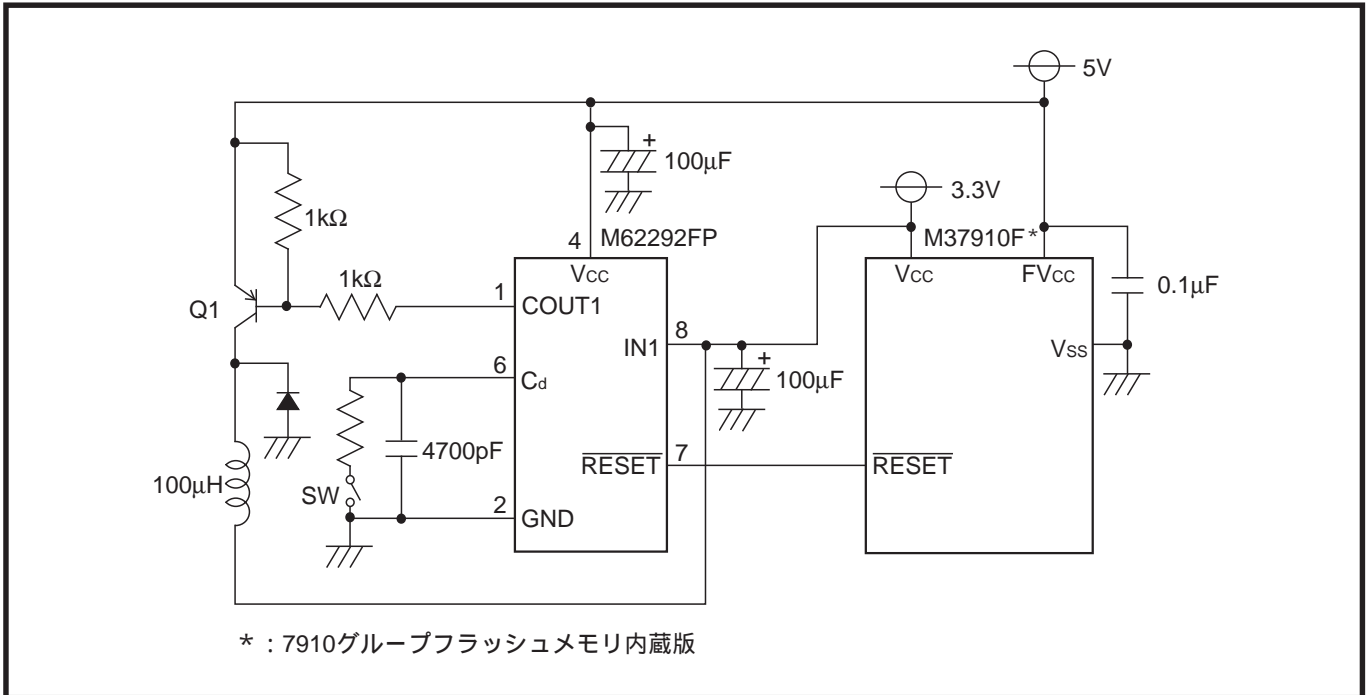
図4.1.4 パワーオンリセット回路例(1)(フラッシュメモリ内蔵版)
