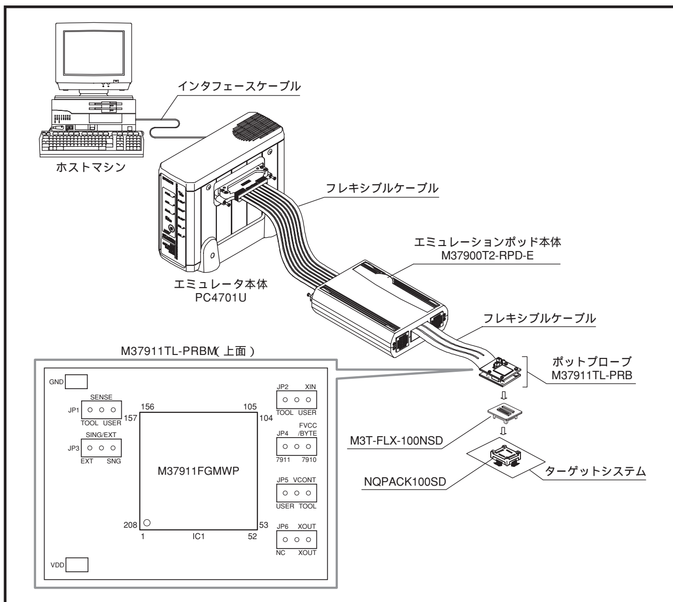
図14 7910グループデバッグ時のシステム構成
