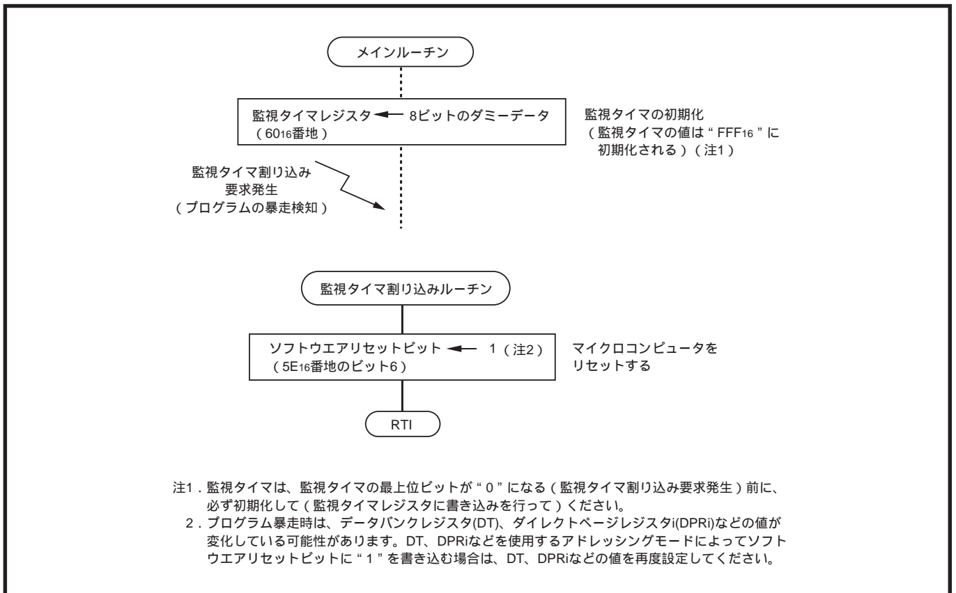
図15.2.1 監視タイマによるプログラムの暴走検知例
