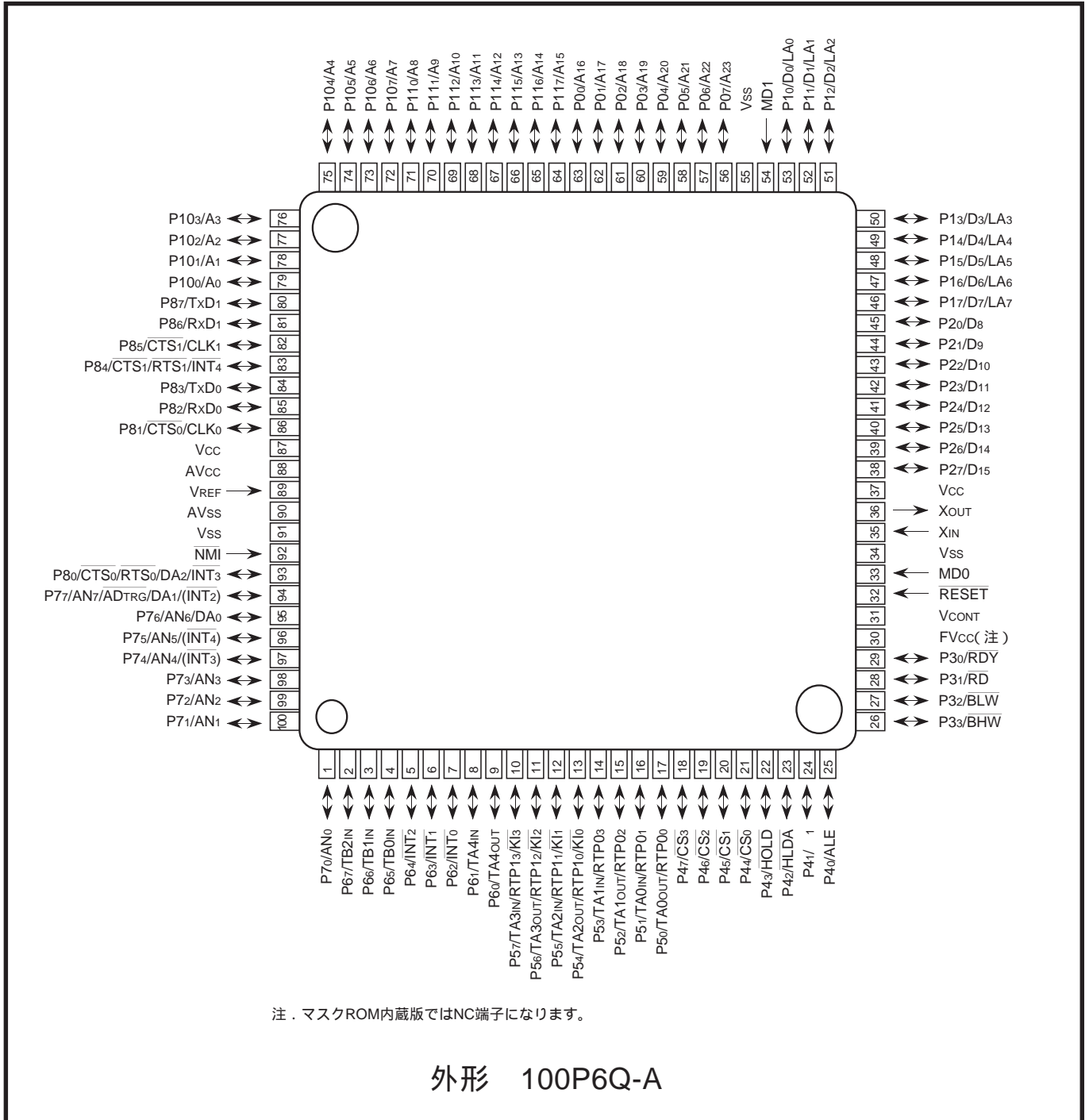
図1.2.1 M37910(外形:100P6Q-A)のピン接続図(上面図)
