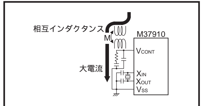
図10 大電流が流れる信号線の配線
