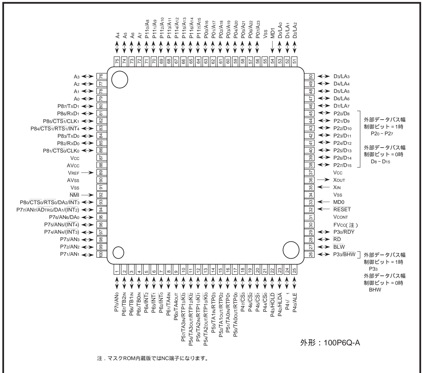
図3.1.1 メモリ拡張モード時のピン接続図(上面図)
