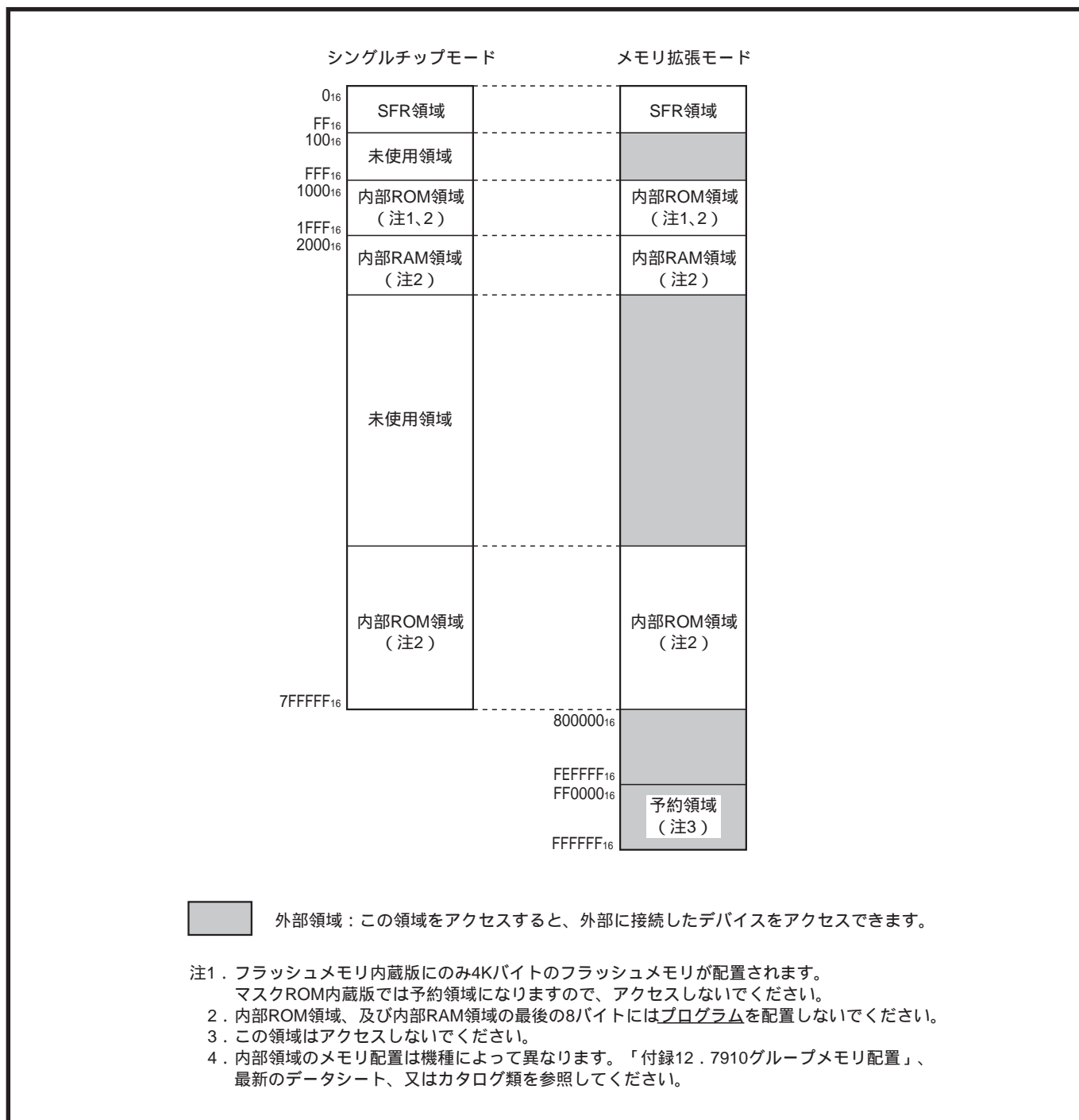
図2.5.1 M37910の各プロセッサモード時のメモリ配置図
