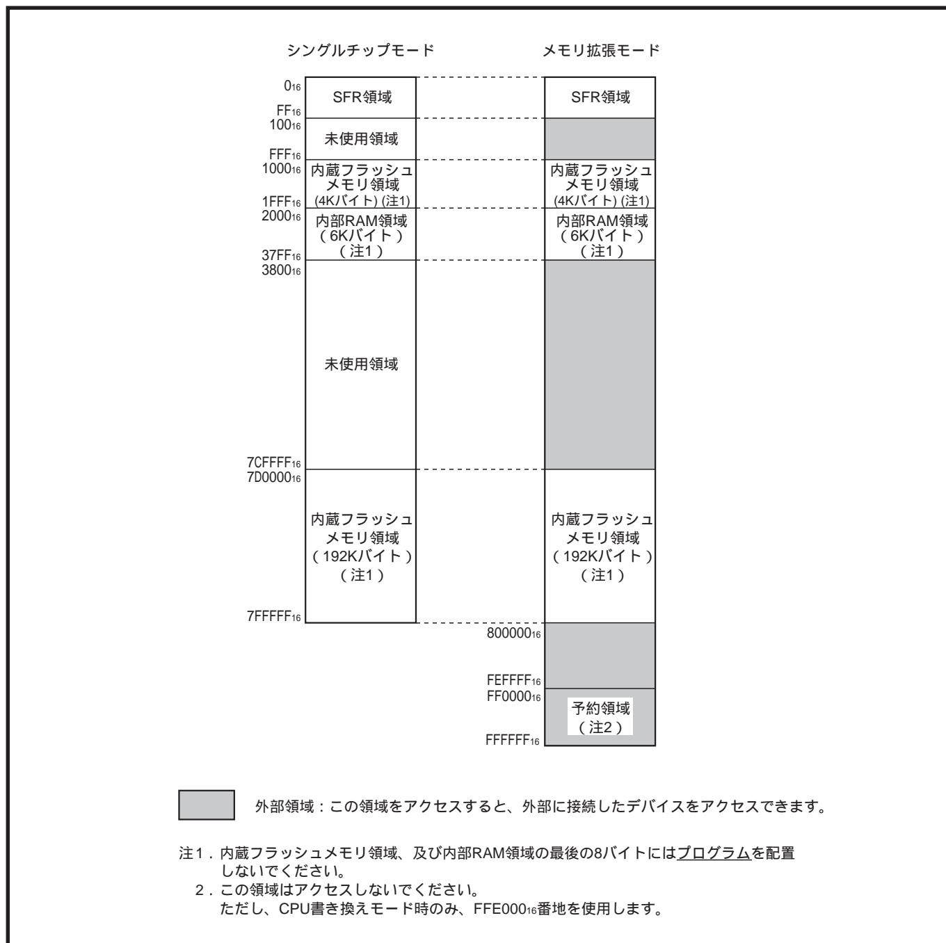
図17 M37910FEMHPのメモリ配置
