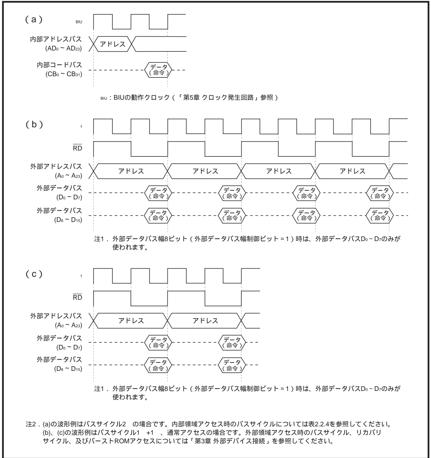
図2.2.3 命令先取り時の動作波形例
