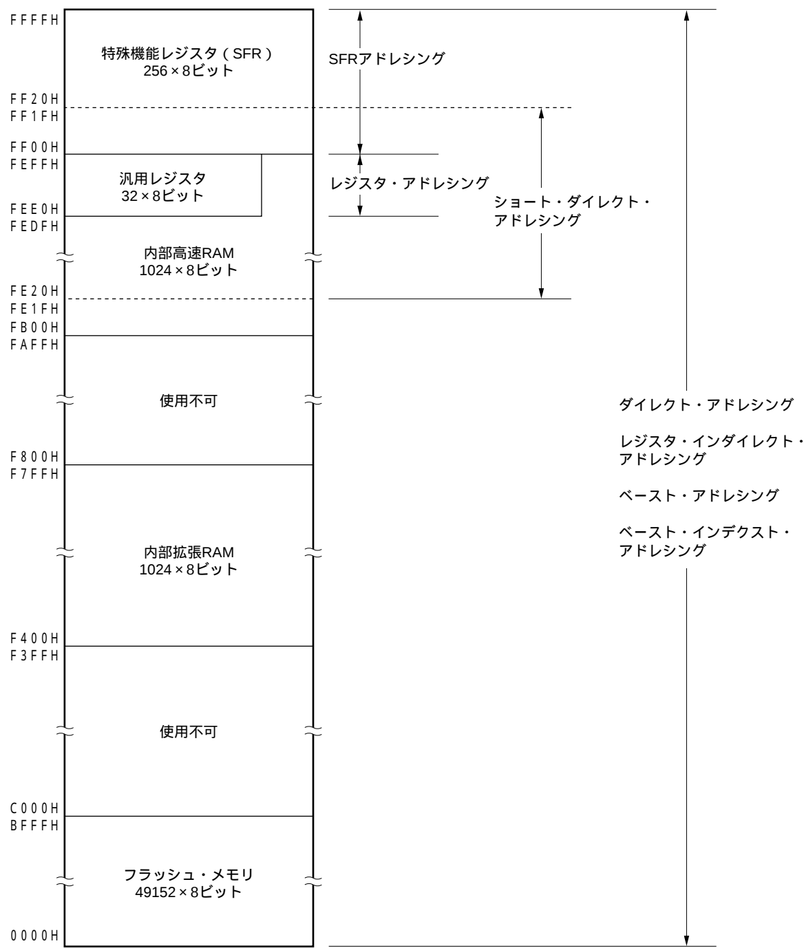
図3 - 10 データ・メモリとアドレッシングの対応 (μ PD78F0136H)
