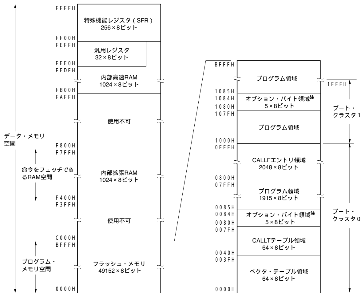
図3 - 4 メモリ・マップ (μPD78F0136H)
