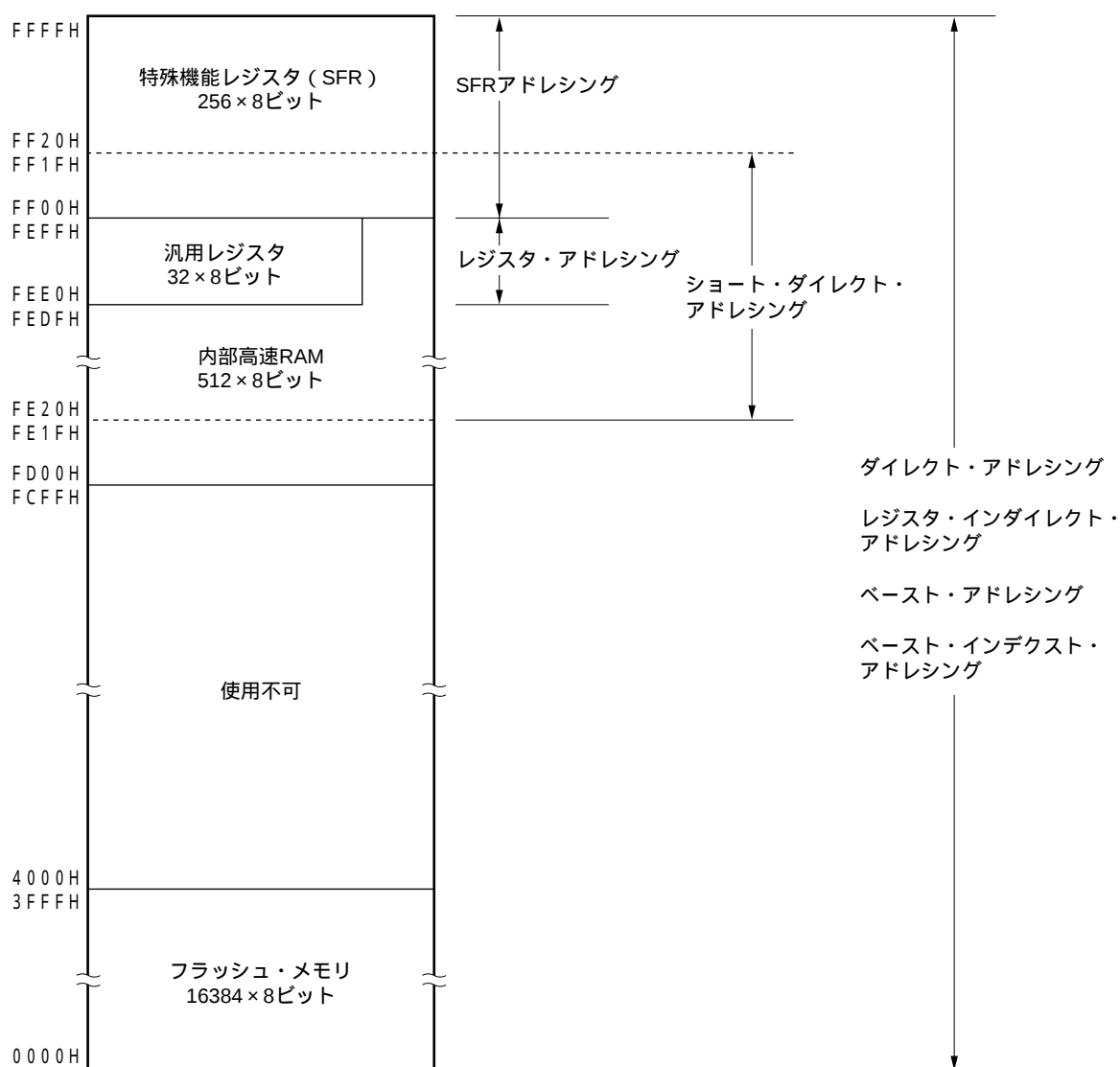
図3-7 データ・メモリとアドレッシングの対応 (μ PD78F0132H)
