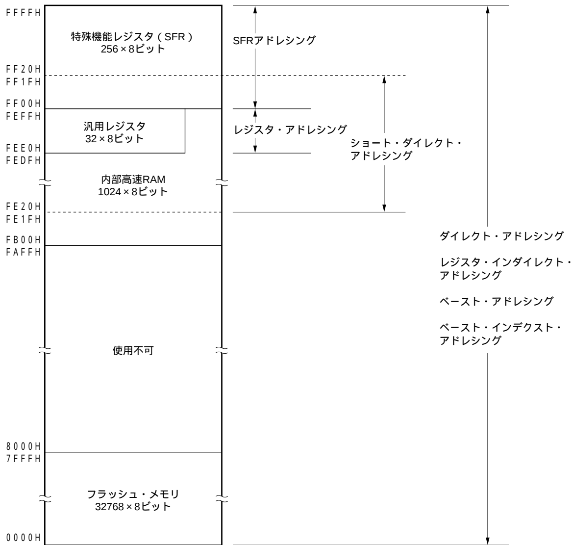
図3 - 9 データ・メモリとアドレッシングの対応 (μ PD78F0134H)
