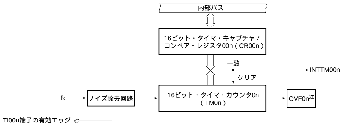
図6 - 32 外部イベント・カウンタの構成図
