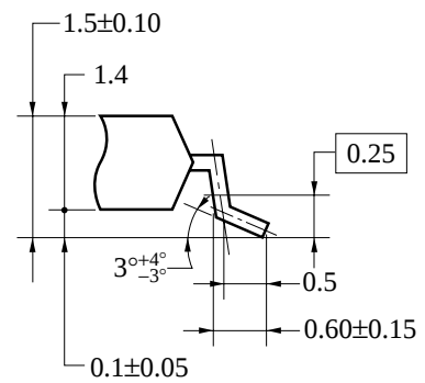
端子先端形状詳細図
