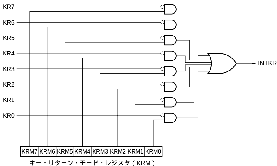
図18 - 1 キー割り込みのブロック図
