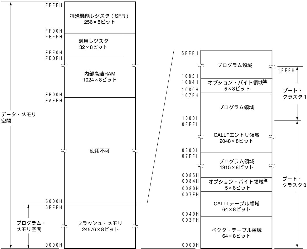
図3 - 2 メモリ・マップ (μPD78F0133H)
