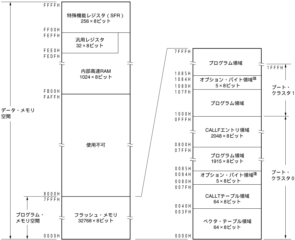
図3 - 3 メモリ・マップ (μPD78F0134H)
