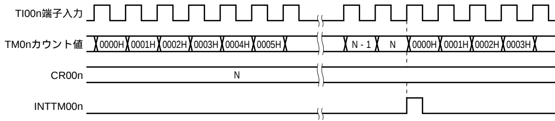
図6 - 33 外部イベント・カウンタ動作のタイミング（立ち上がりエッジ指定時）
