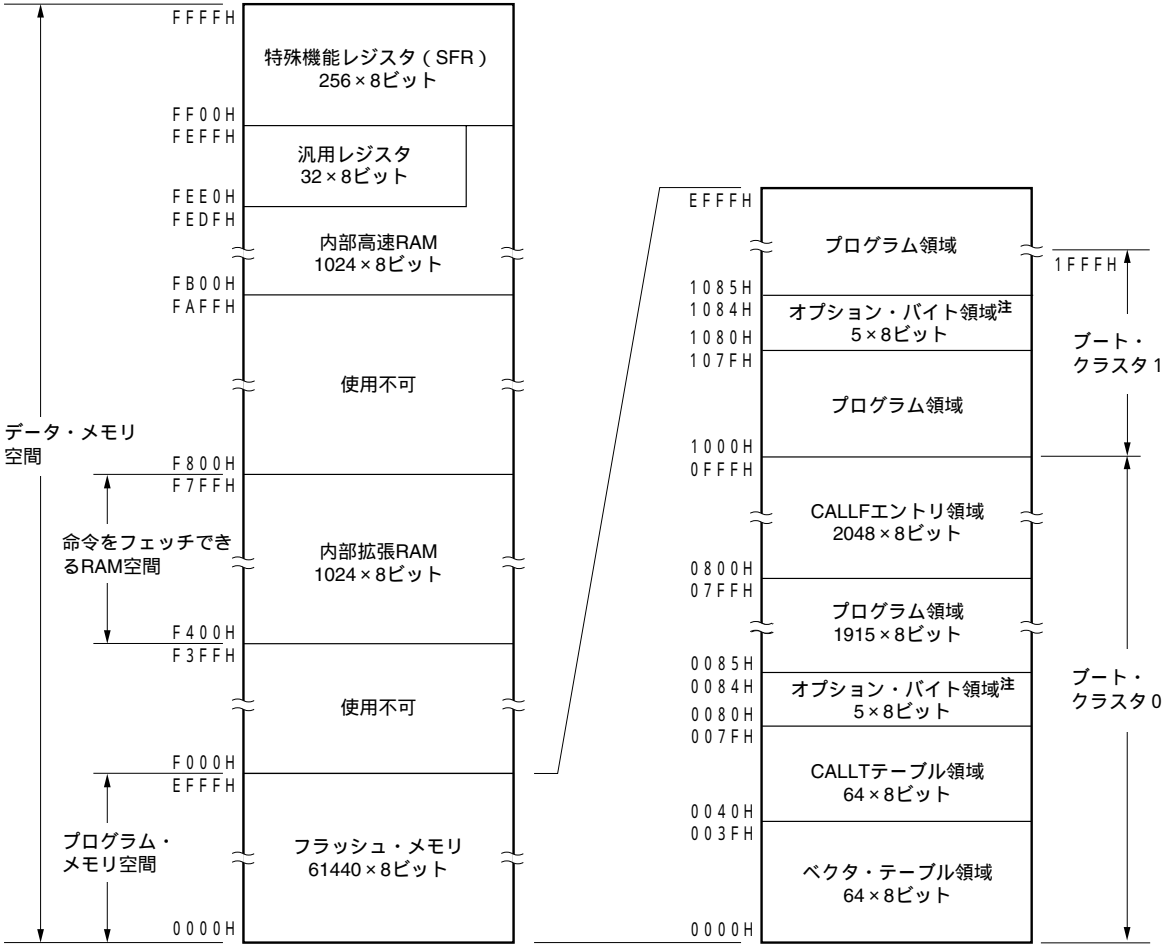
図3 - 5 メモリ・マップ (μPD78F0138H)
