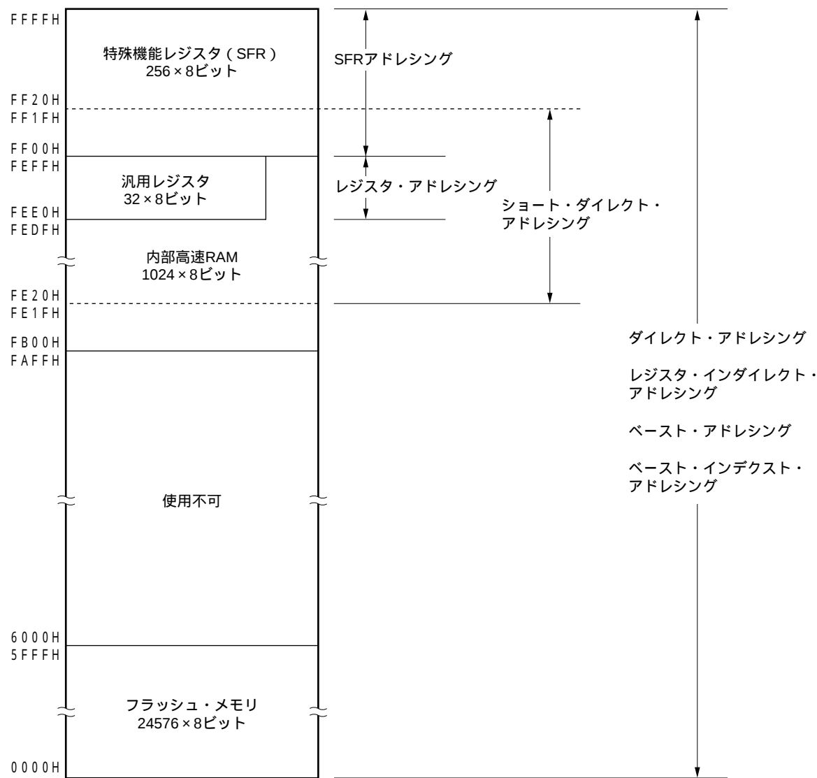
図3 - 8 データ・メモリとアドレッシングの対応 (μ PD78F0133H)
