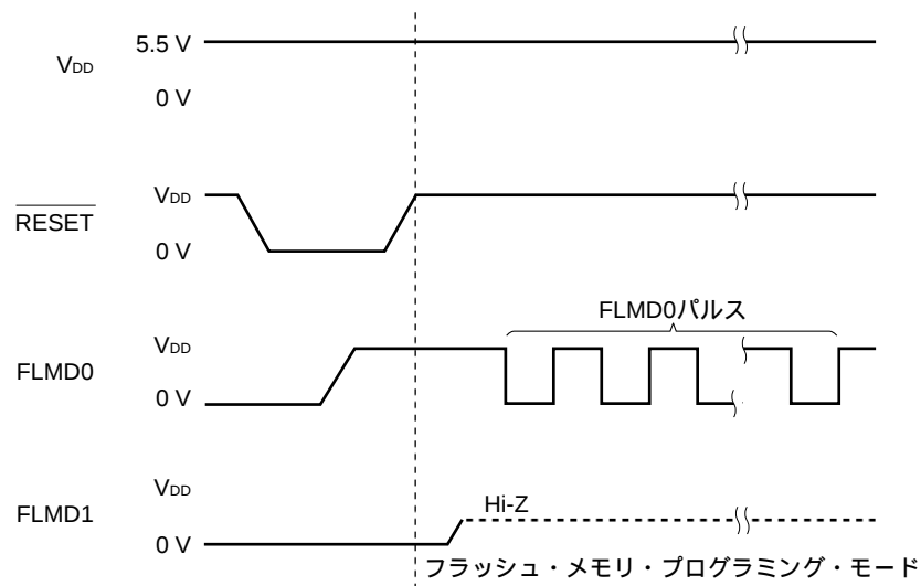
図26 - 16 フラッシュ・メモリ・プログラミング・モード
