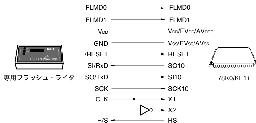
図26 - 8 専用フラッシュ・ライタとの通信 (CSI10 + HS)
