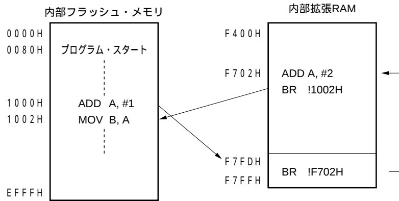
図25 - 4 ROMコレクションの使用例
