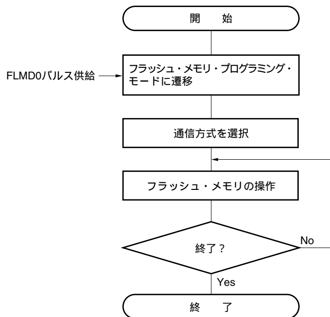
図26 - 15 フラッシュ・メモリの操作手順
