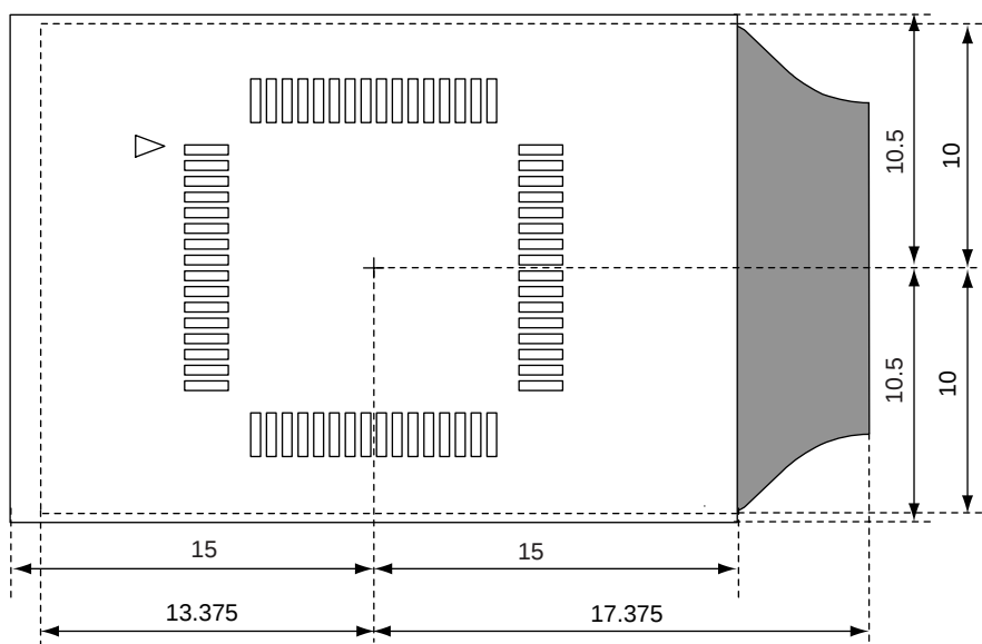
図B - 2 ターゲット・システム上の制限領域 (64ピンGKパッケージの場合)
