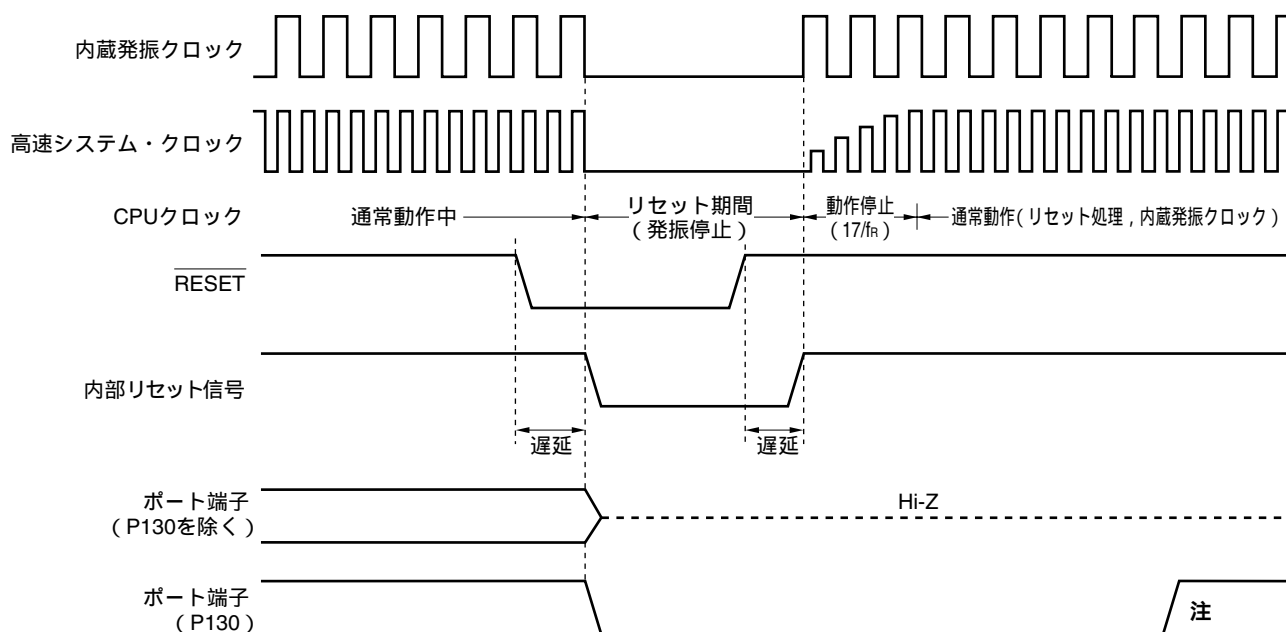
図20 - 2 RESET入力によるリセット・タイミング
