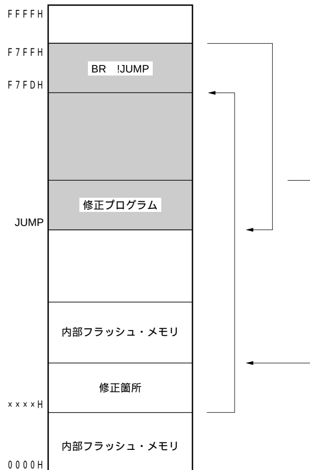
図25 - 8 プログラム遷移図（修正箇所が1つの場合）
