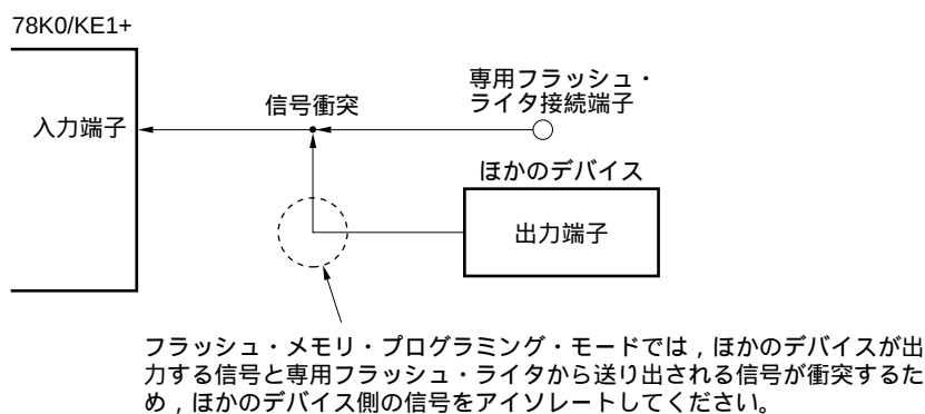
図26 - 12 信号の衝突（シリアル・インタフェースの入力端子）
