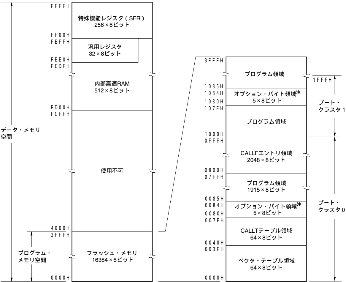
図3 - 1 メモリ・マップ (μPD78F0132H)
