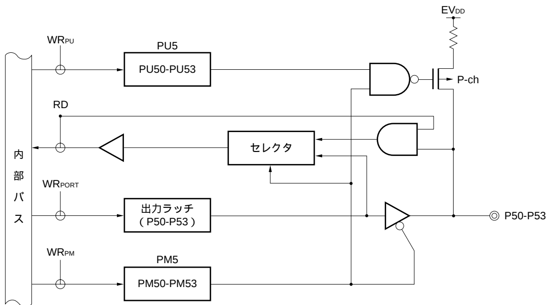
図4 - 15 P50-P53のブロック図
