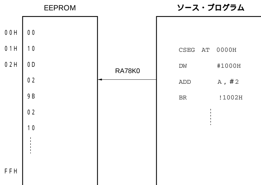
図25 - 5 EEPROMへの格納例 (修正箇所が1つの場合)
