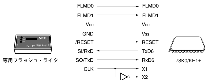
図26 - 9 専用フラッシュ・ライタとの通信 (UART6)
