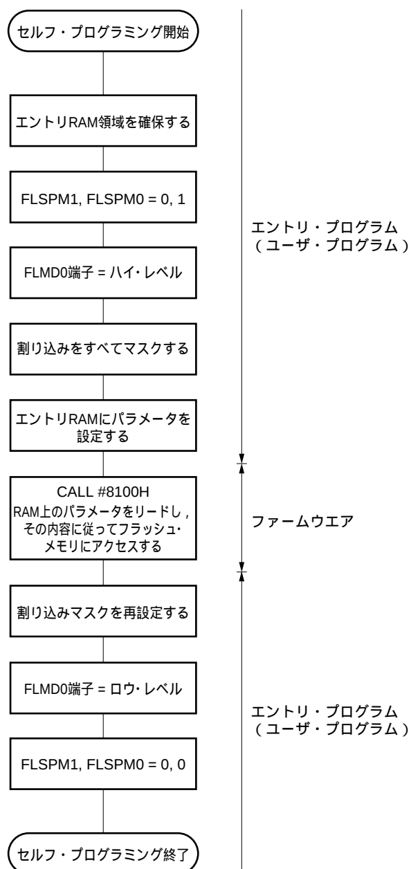
図26 - 18 セルフ・プログラミングの手順
