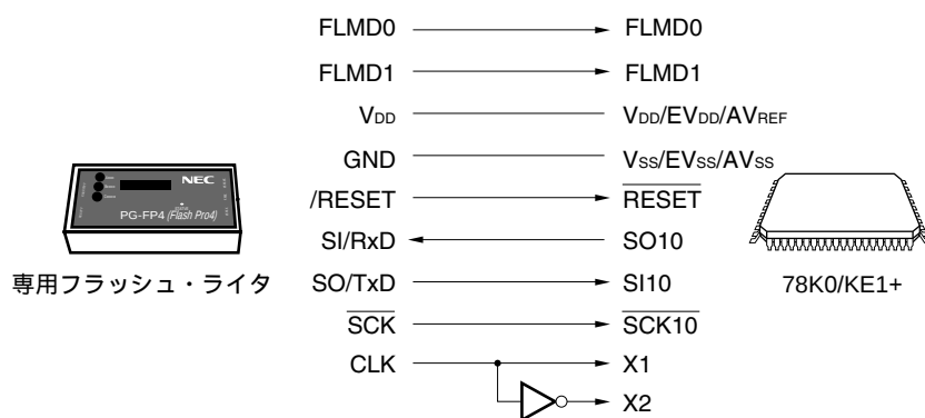
図26 - 7 専用フラッシュ・ライターとの通信 (CSI10)
