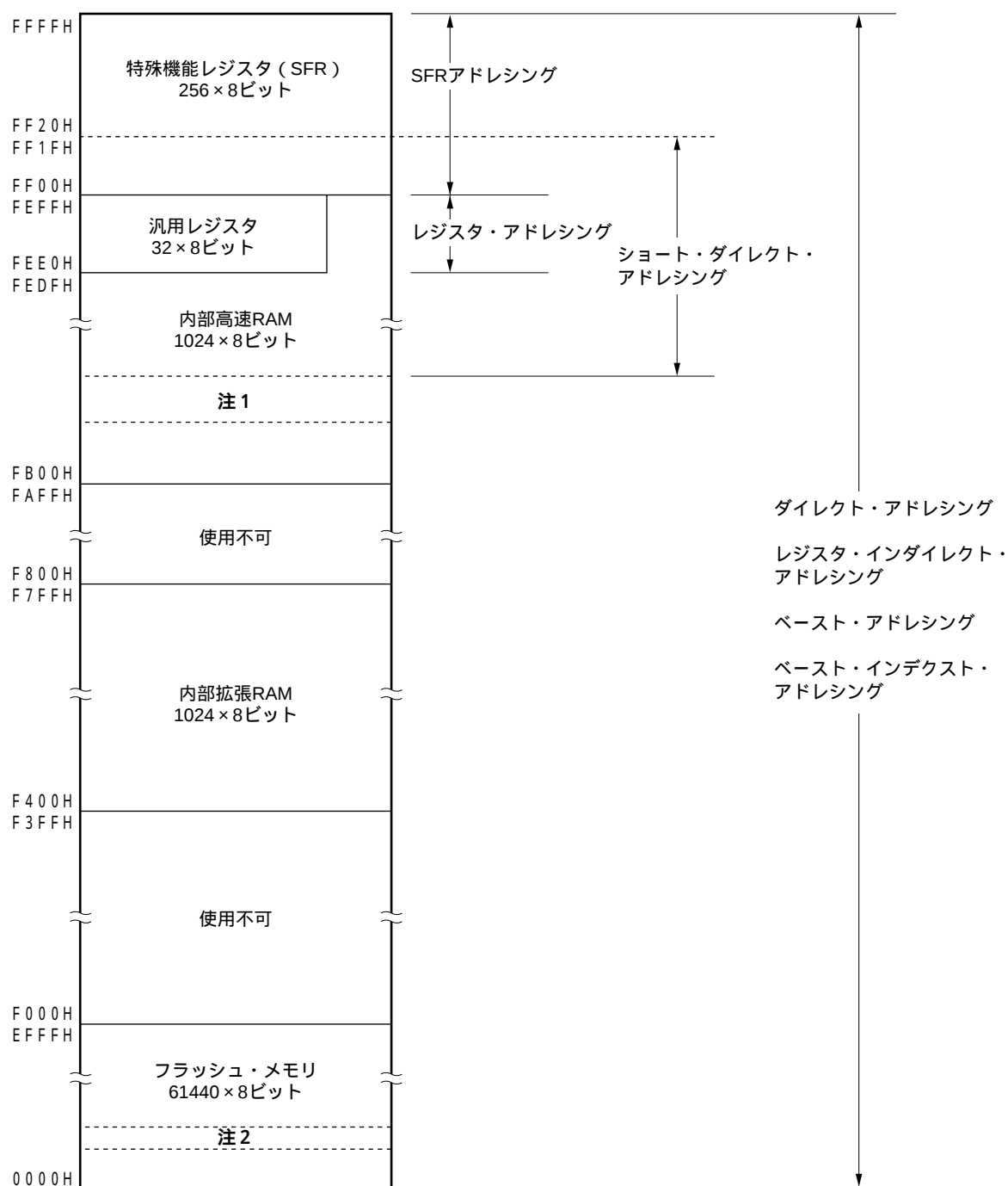
図3 - 12 データ・メモリとアドレッシングの対応 (μ PD78F0138HD)
