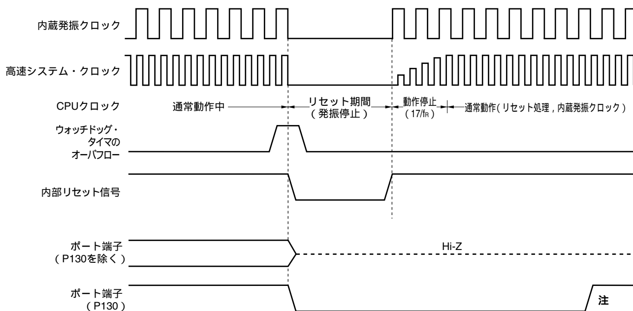
図20 - 3 ウォッチドッグ・タイマのオーバーフローによるリセット・タイミング
