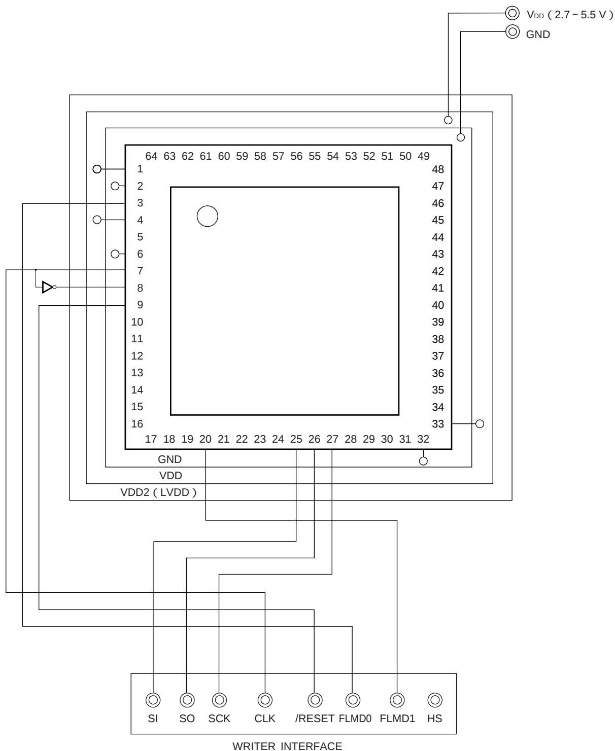
図26 - 3 3線式シリアルI/O (CSI10) 方式でのフラッシュ書き込み用アダプタ配線例
