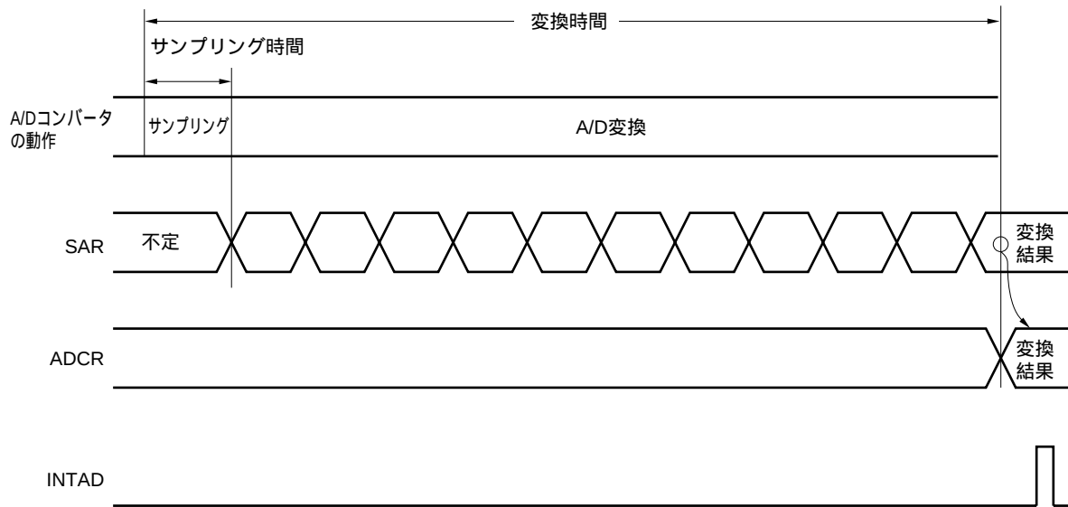
図12 - 9 A/Dコンバータの基本動作
