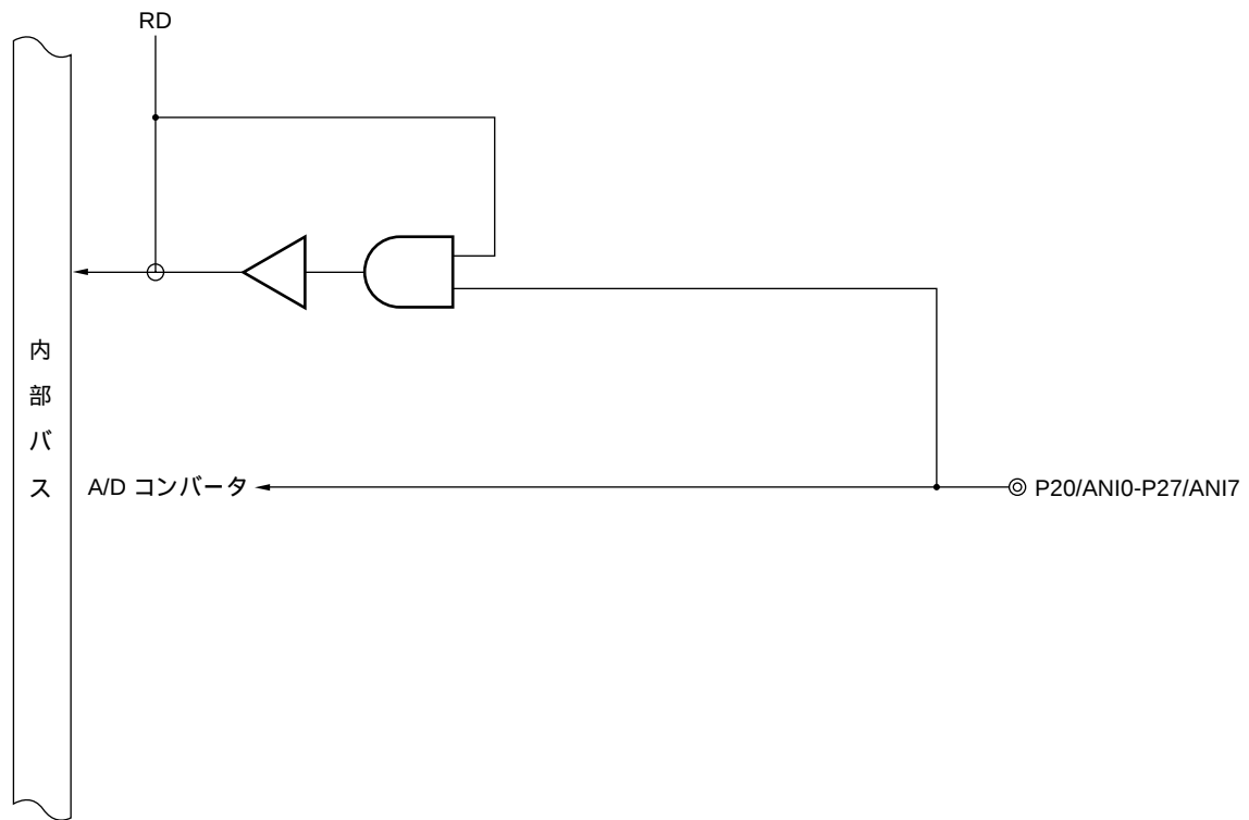
図4 - 11 P20-P27のブロック図
