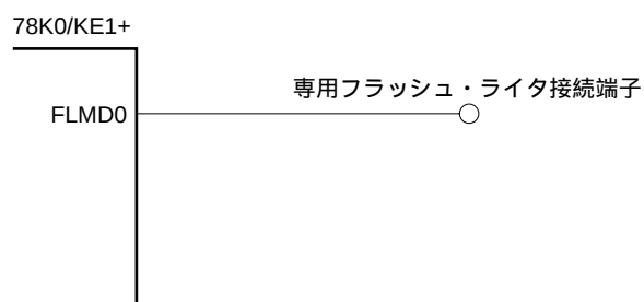
図26 - 10 FLMD0端子の接続例
