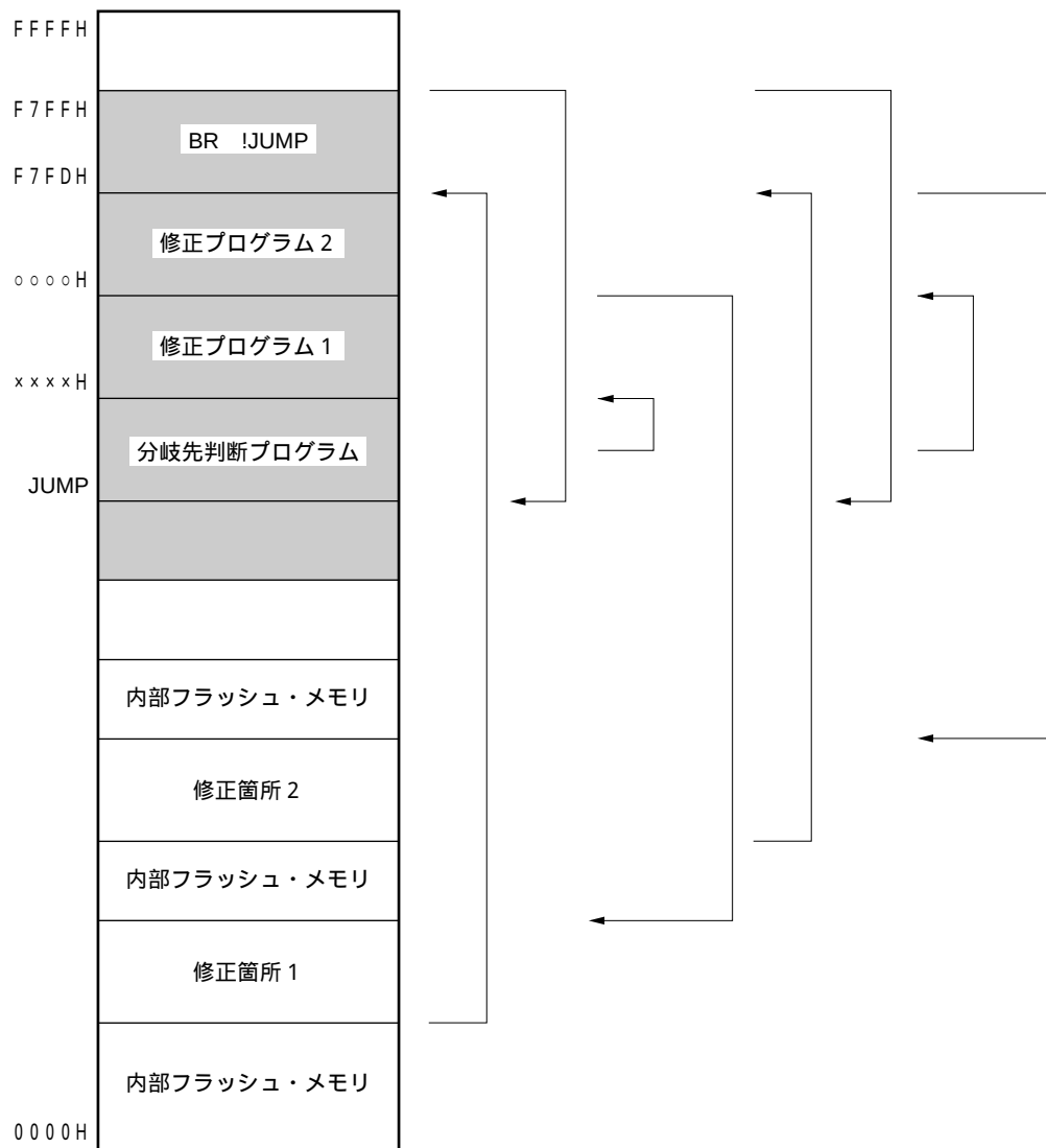
図25 - 9 プログラム遷移図（修正箇所が2つの場合）
