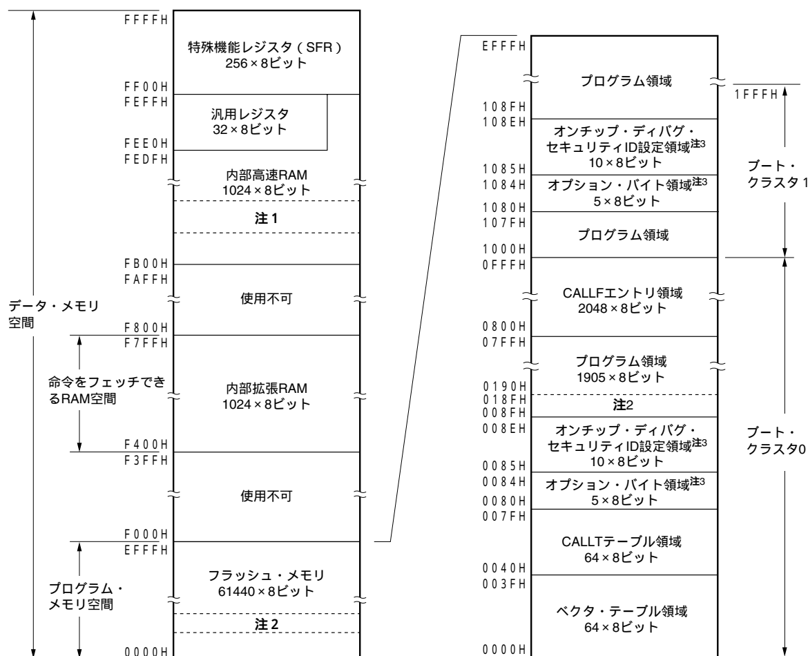
図3-6 メモリ・マップ(μ PD78F0138HD)
