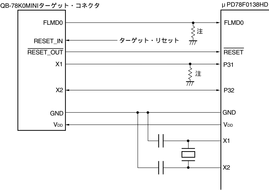
図27 - 2 QB-78K0MINIとμ PD78F0138HDの接続例 (P31, P32使用時)
