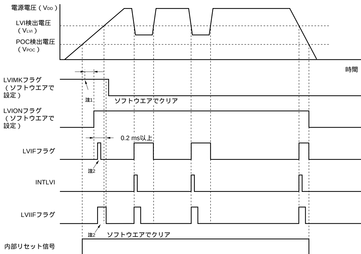
図23 - 5 低電圧検出回路の割り込み信号発生タイミング
