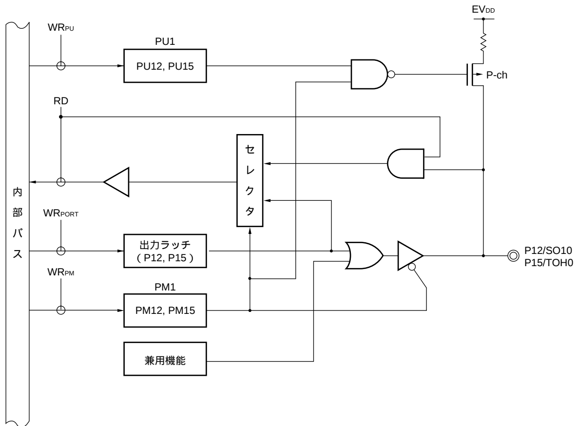
図4 - 8 P12, P15のブロック図
