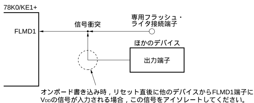
図26 - 11 FLMD1端子の接続例
