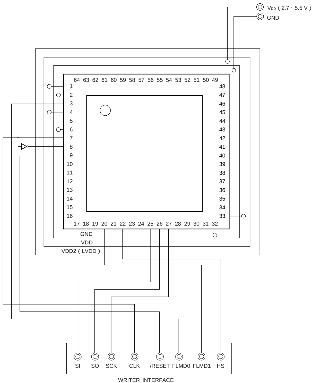
図26 - 4 3線式シリアルI/O (CSI10 + HS) 方式でのフラッシュ書き込み用アダプタ配線例
