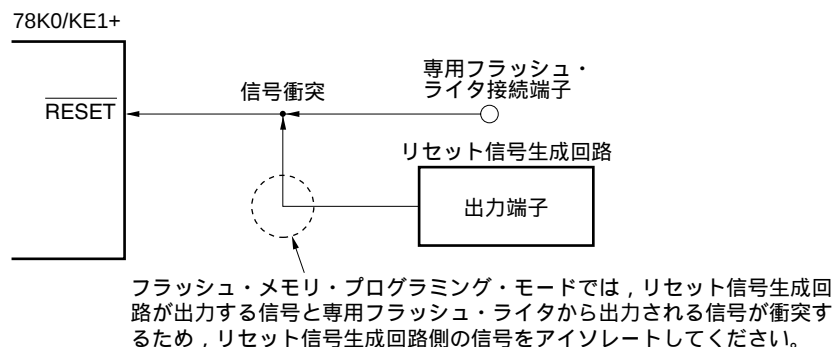
図26 - 14 信号の衝突 (RESET端子)
