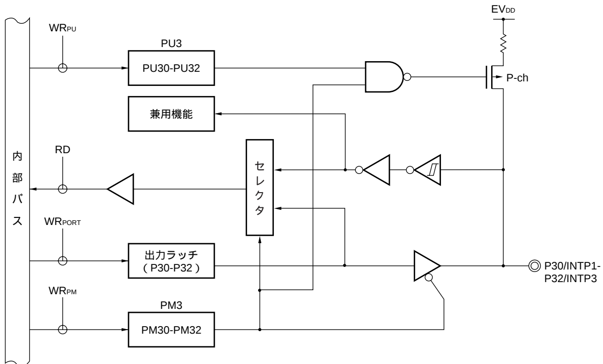
図4 - 12 P30-P32のブロック図
