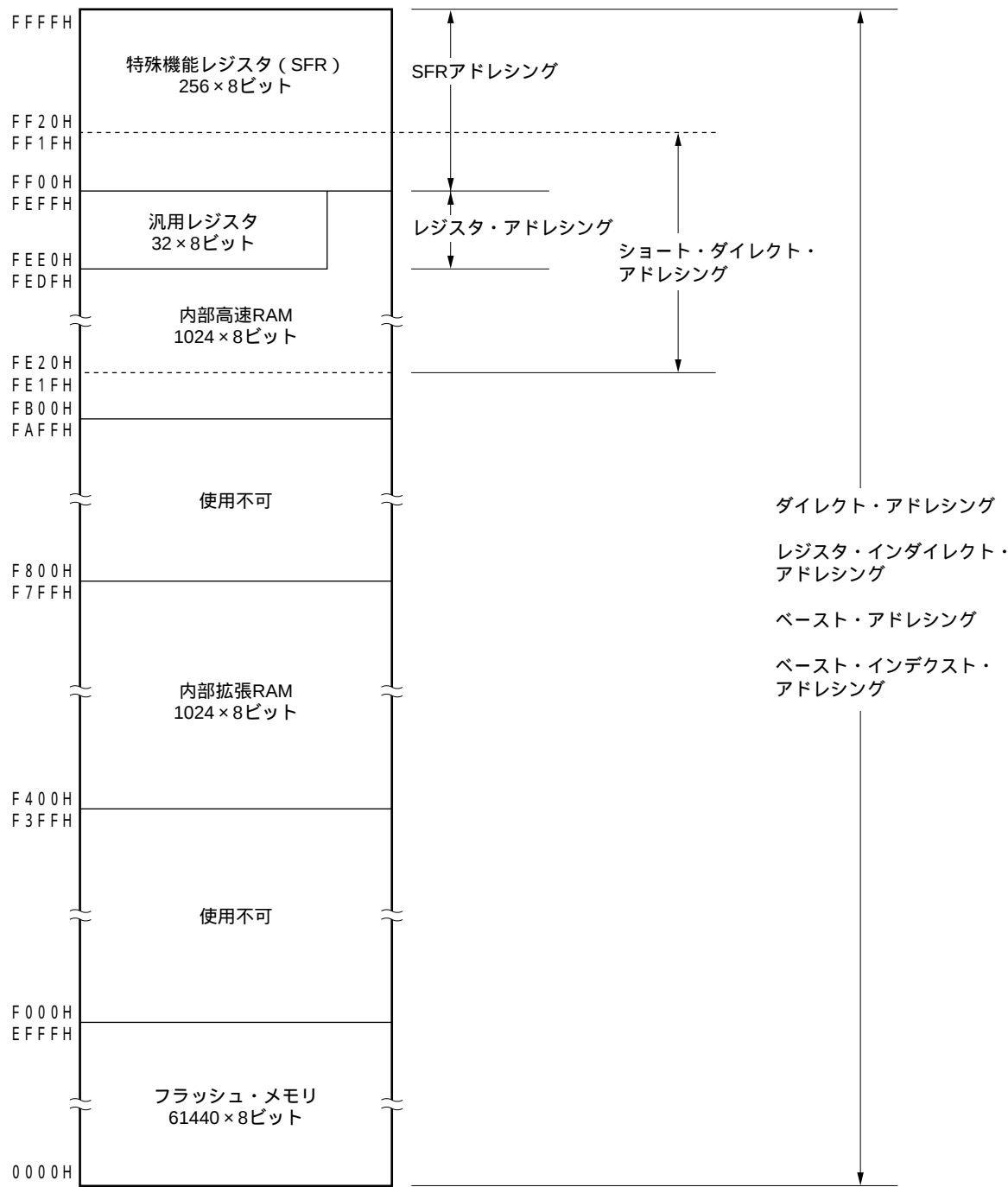
図3 - 11 データ・メモリとアドレッシングの対応 (μ PD78F0138H)
