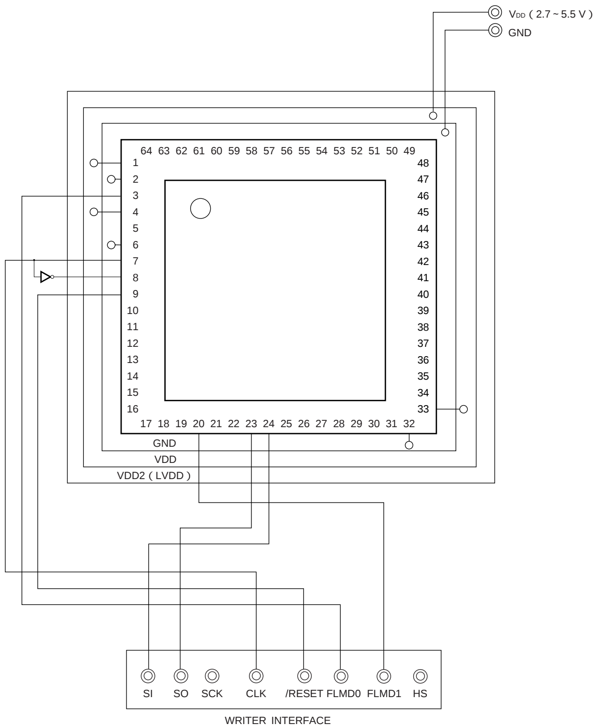
図26 - 5 UART (UART6) 方式でのフラッシュ書き込み用アダプタ配線例
