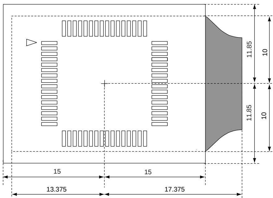
図B - 3 ターゲット・システム上の制限領域 (64ピンGCパッケージの場合)
