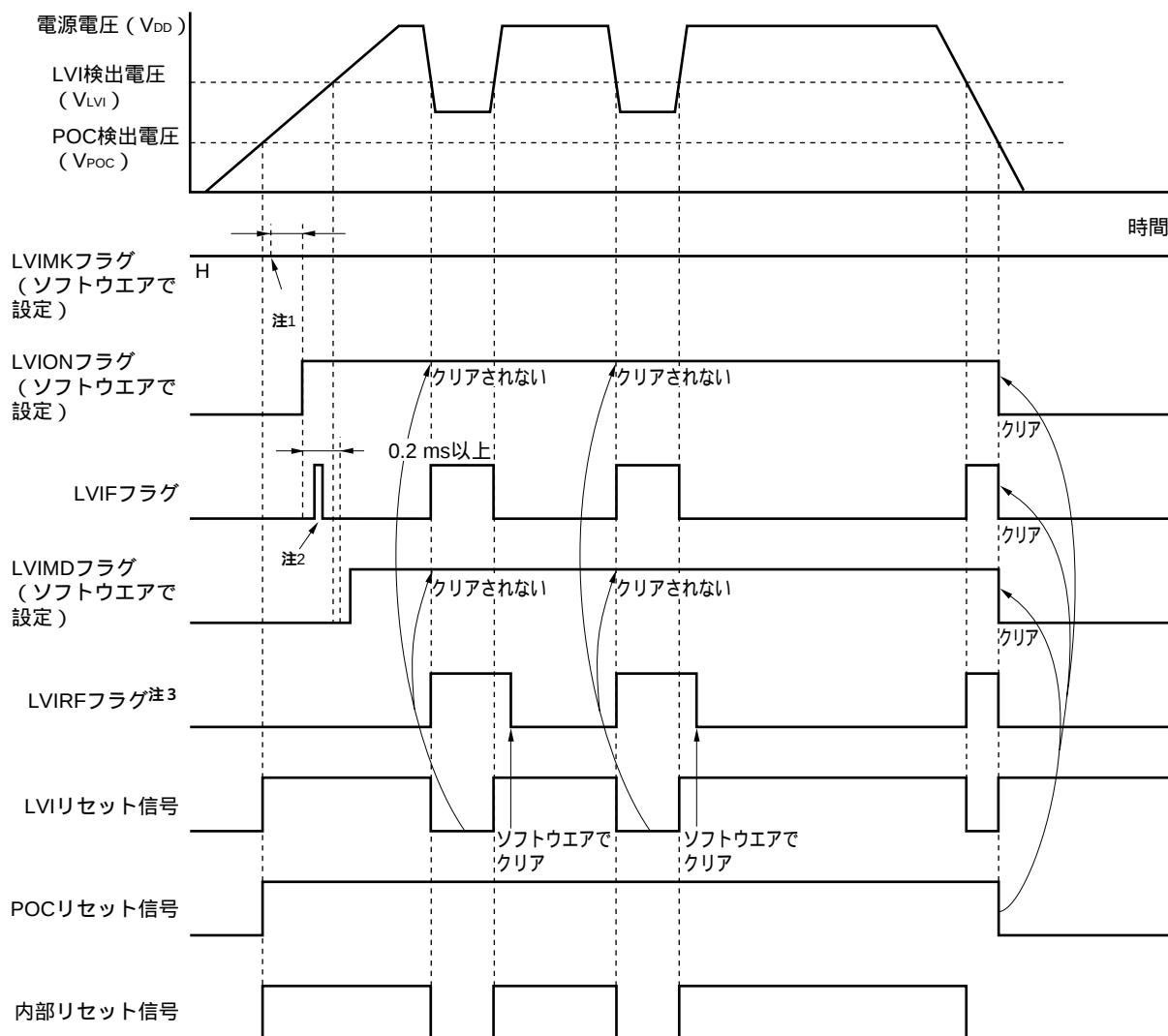
図23 - 4 低電圧検出回路の内部リセット信号発生タイミング
