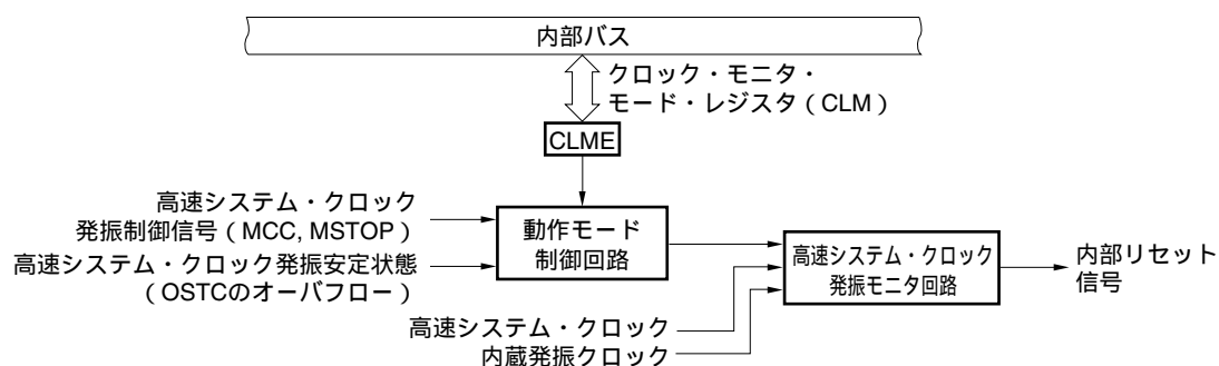
図21-1 クロック・モニタのブロック図
