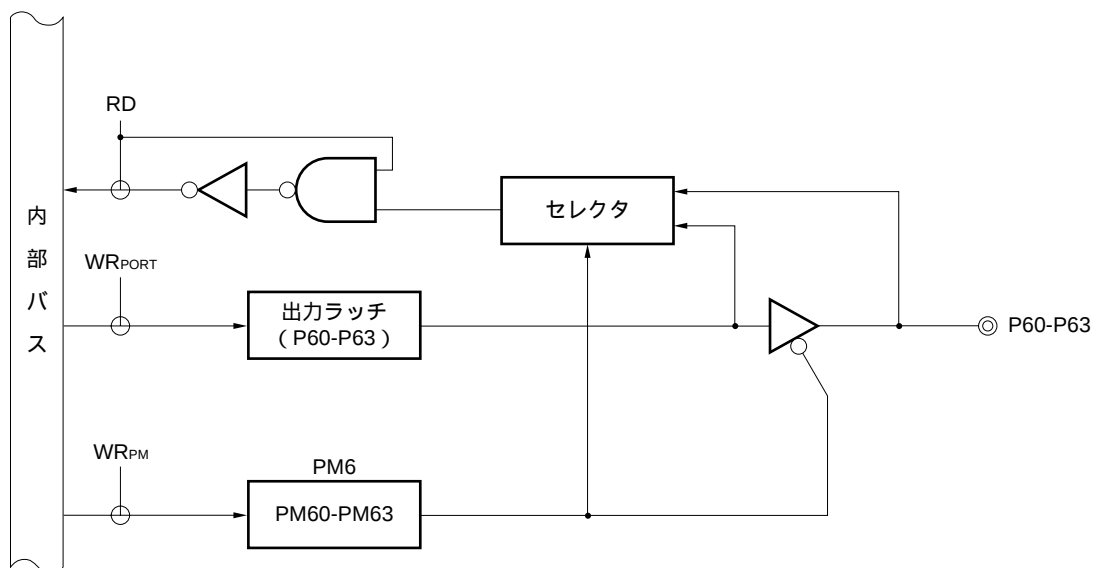
図4 - 16 P60-P63のブロック図
