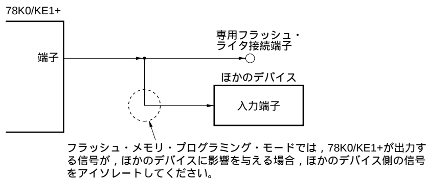
図26 - 13 ほかのデバイスの異常動作
