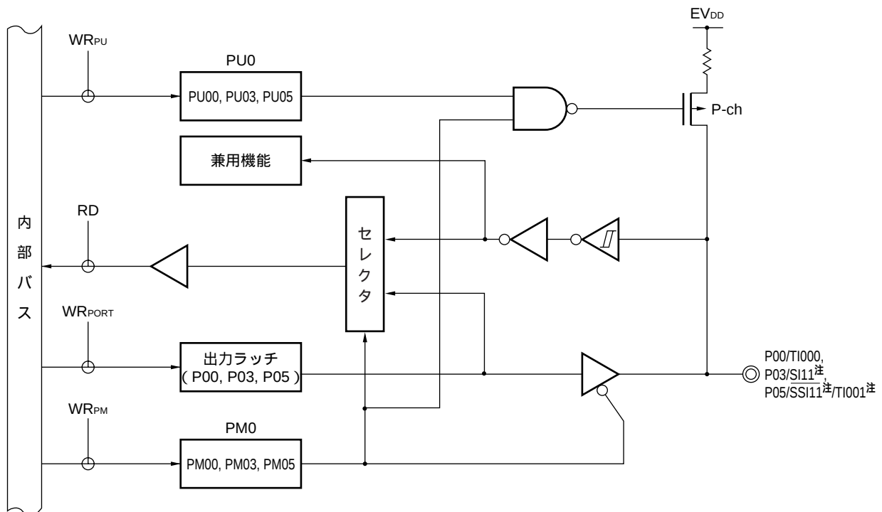
図4 - 2 P00, P03, P05のブロック図
