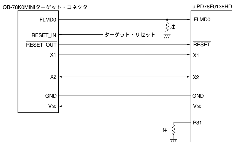
図27 - 1 QB-78K0MINIと \mu PD78F0138HDの接続例 (X1, X2使用時)
