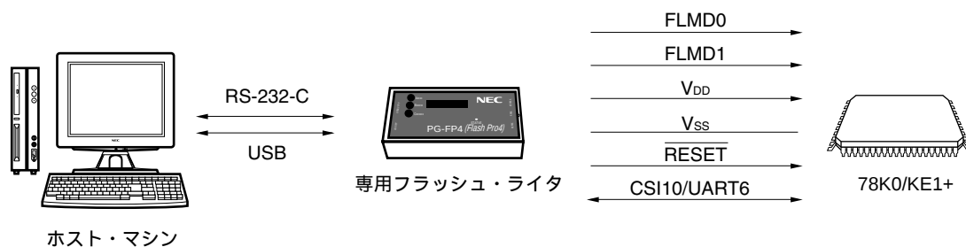
図26 - 6 フラッシュ・メモリにプログラムを書き込むための環境
