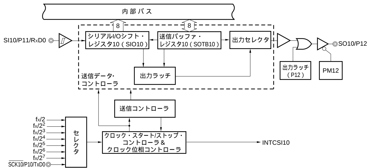
図15 - 2 シリアル・インタフェースCSI11のブロック図
