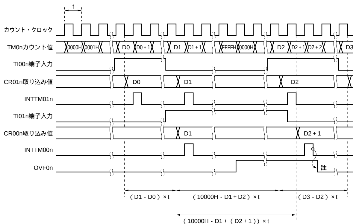
図6 - 26 フリー・ランニング・カウンタによるパルス幅測定動作のタイミング（両エッジ指定時）
