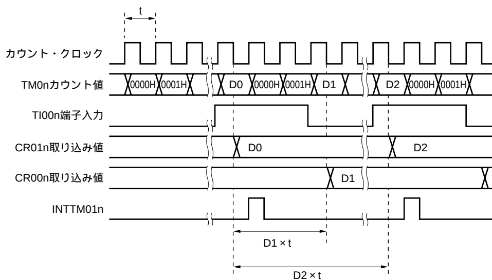
図6 - 30 リスタートによるパルス幅測定動作のタイミング（立ち上がりエッジ指定時）
