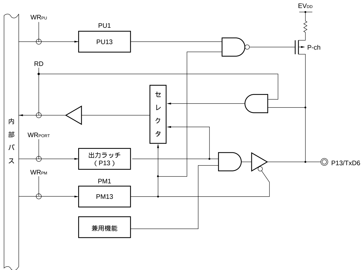
図4 - 9 P13のブロック図
