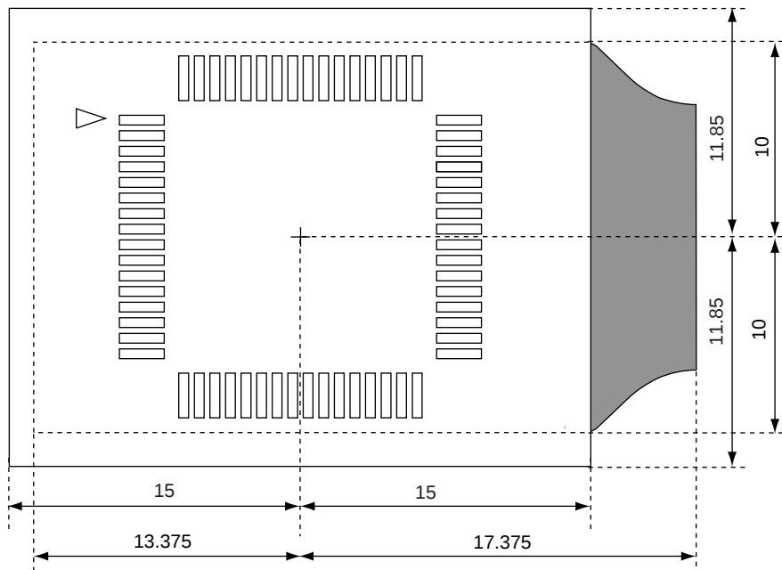
図B - 10 ターゲット・システム上の制限領域 (64ピンGCパッケージの場合)
