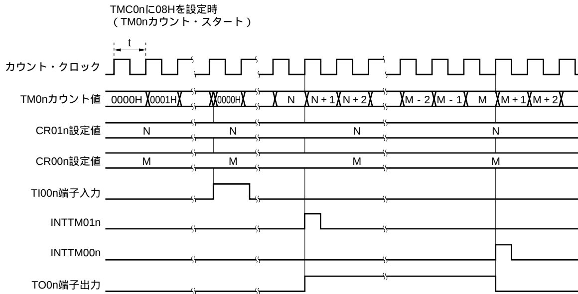
図6 - 39 外部トリガによるワンショット・パルス出力動作のタイミング（立ち上がりエッジ指定時）
