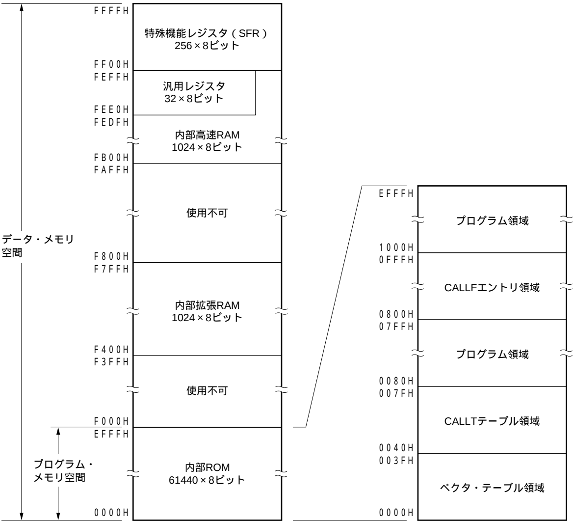
図3 - 7 メモリ・マップ (μPD780138)
