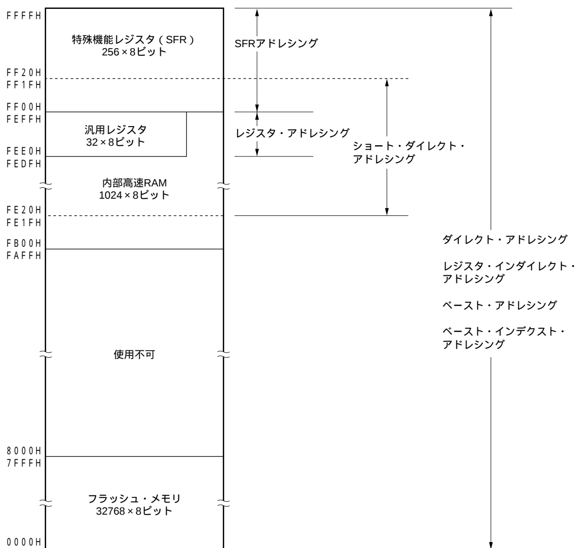
図3 - 13 データ・メモリとアドレッシングの対応 (μ PD78F0134)
