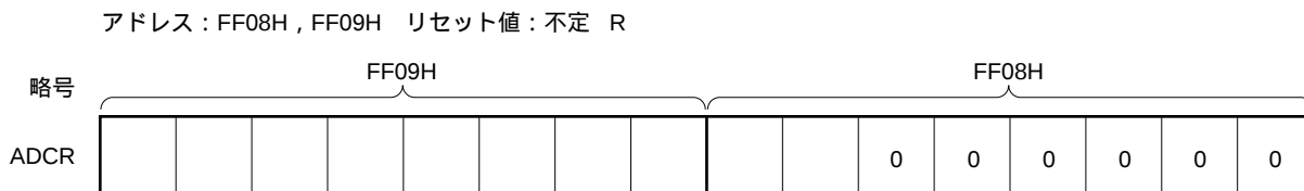
図12 - 6 A/D変換結果レジスタ (ADCR) のフォーマット
