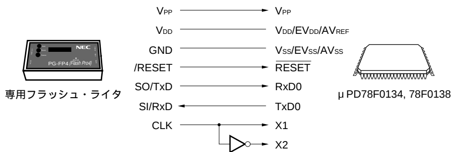
図27 - 11 専用フラッシュ・ライタとの通信 (UART0)
