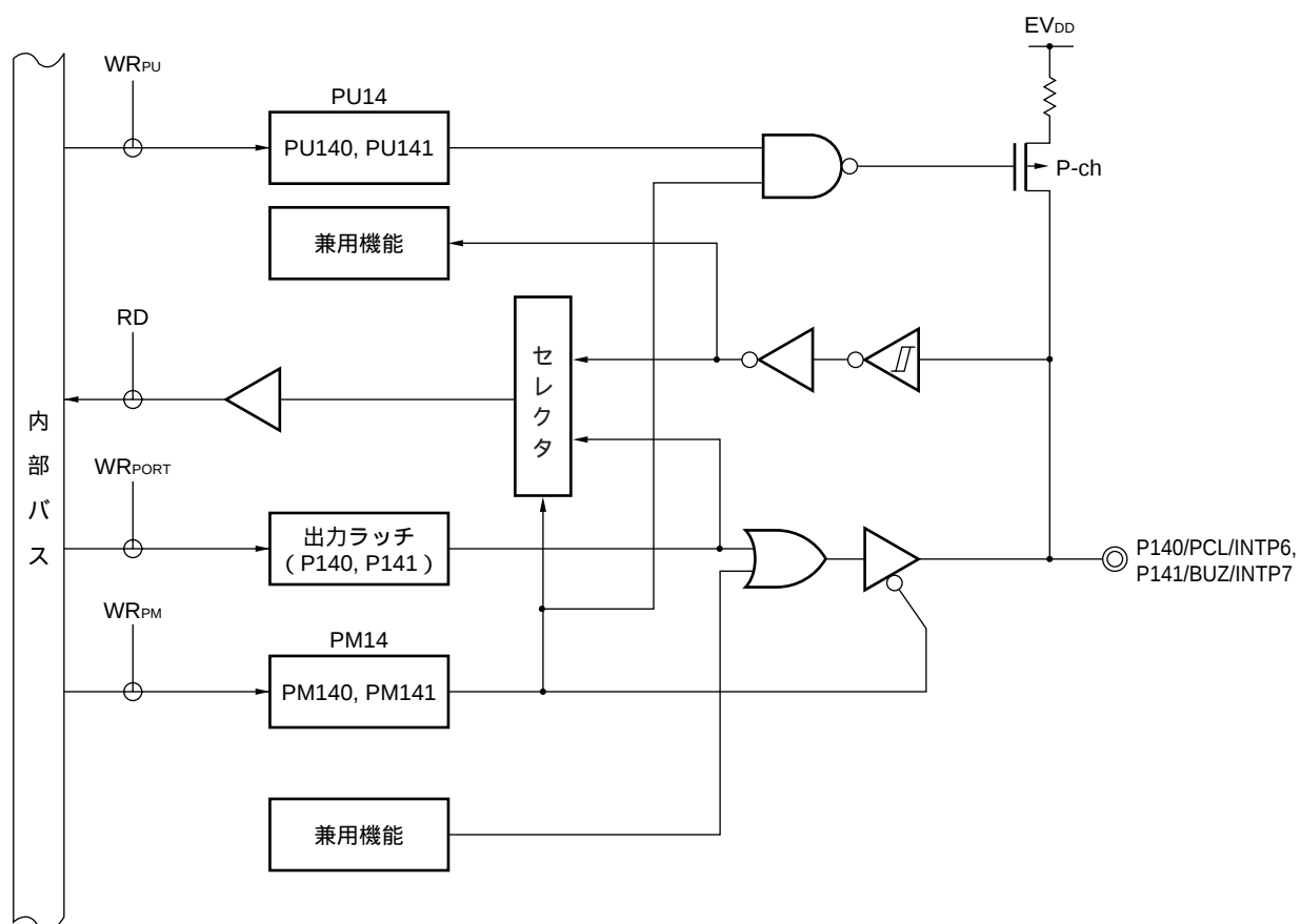
図4 - 20 P140, P141のブロック図
