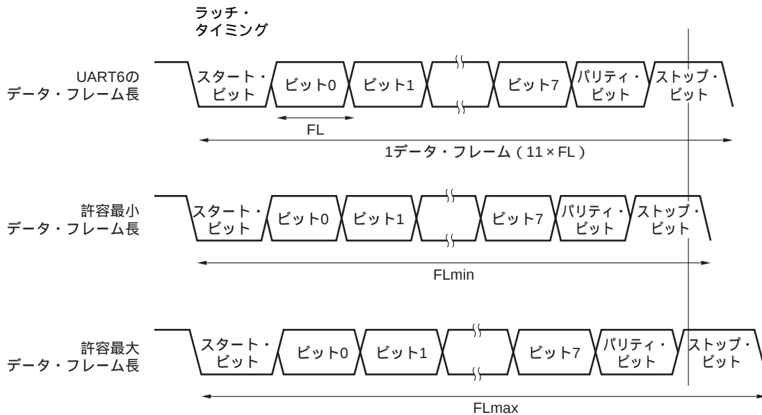
図14 - 26 受信時の許容ボー・レート範囲
