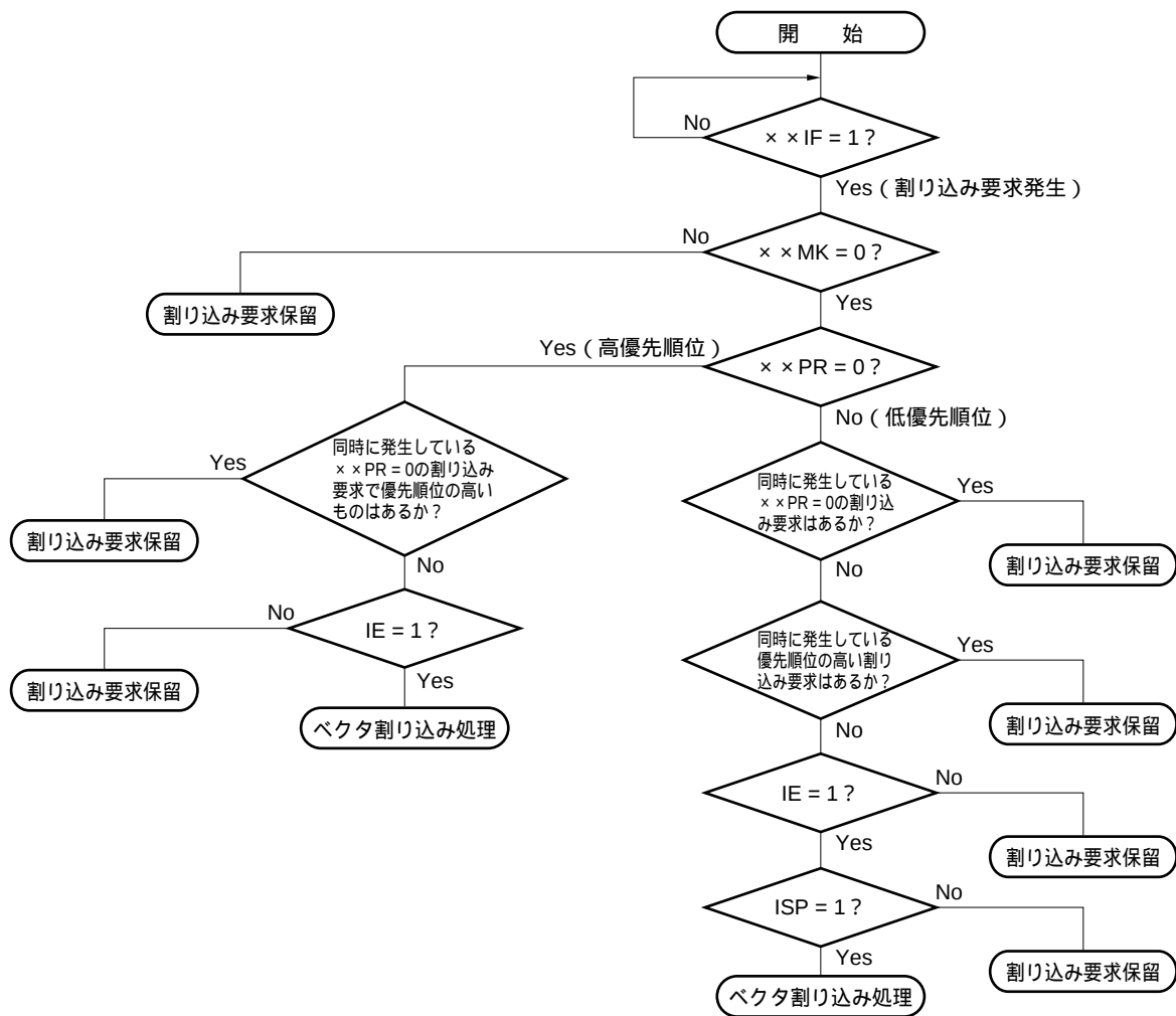
図17-7 割り込み要求受け付け処理アルゴリズム
