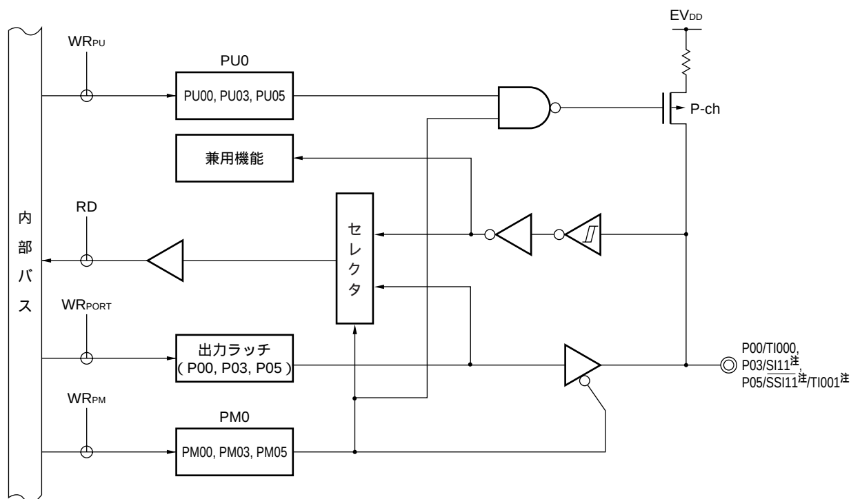
図4 - 2 P00, P03, P05のブロック図
