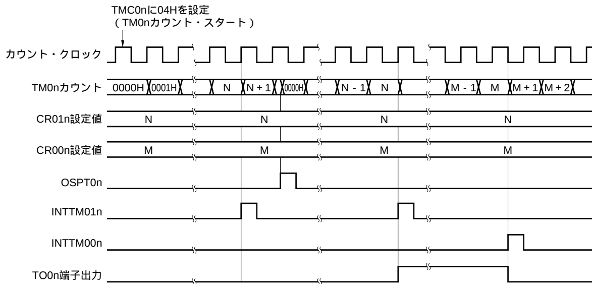
図6 - 37 ソフトウェア・トリガによるワンショット・パルス出力動作のタイミング
