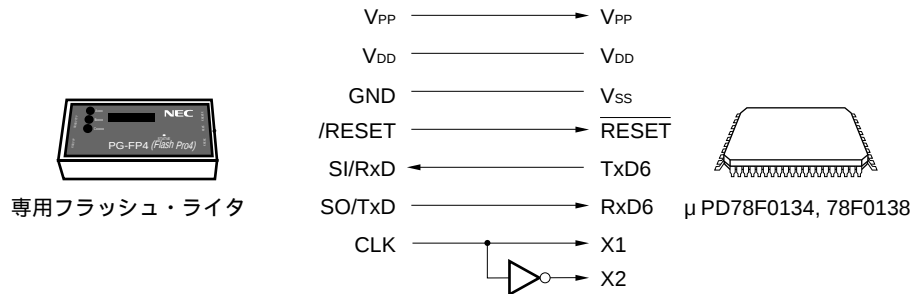
図27 - 13 専用フラッシュ・ライタとの通信 (UART6)
