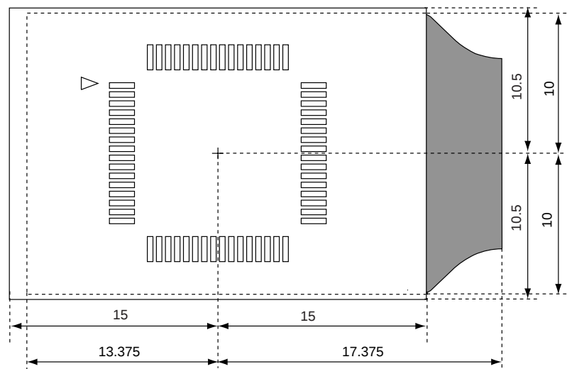
図B - 9 ターゲット・システム上の制限領域 (64ピンGKパッケージの場合)
