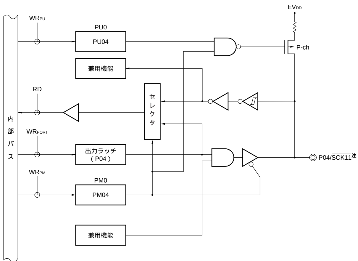
図4 - 5 P04のブロック図
