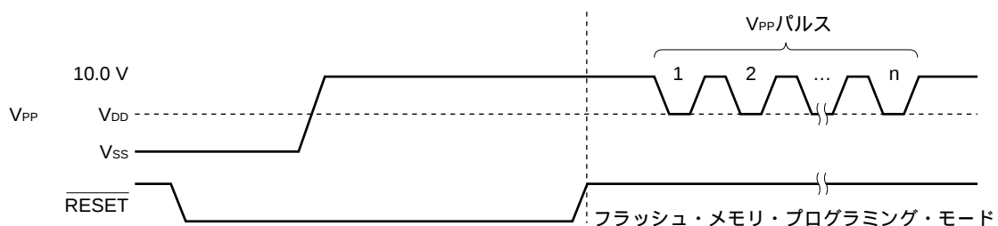
図27 - 19 フラッシュ・メモリ・プログラミング・モード
