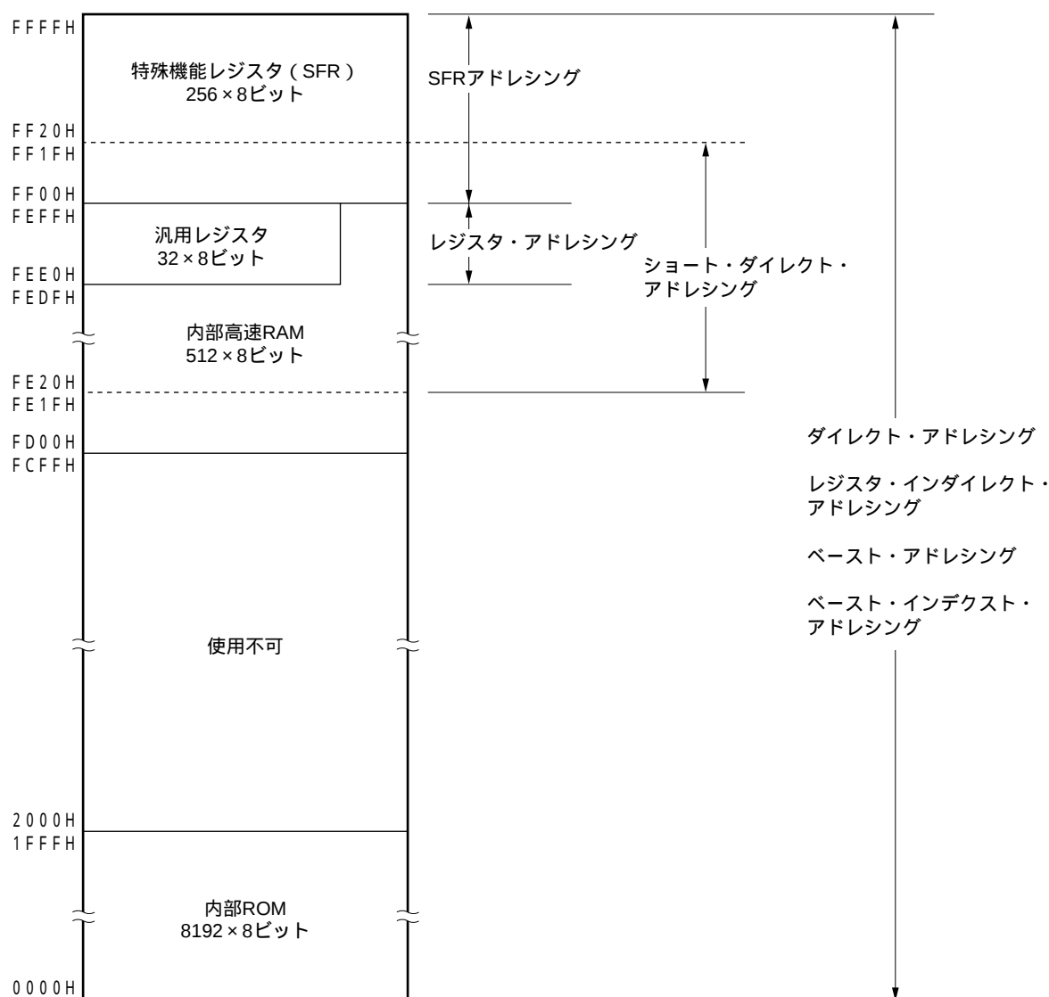
図3 - 9 データ・メモリとアドレッシングの対応 (μ PD780131)
