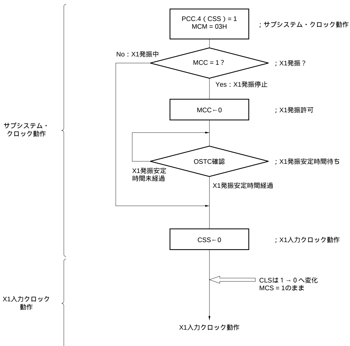
図5 - 17 サブシステム・クロックからX1入力クロックへの切り替え (フロー・チャート)
