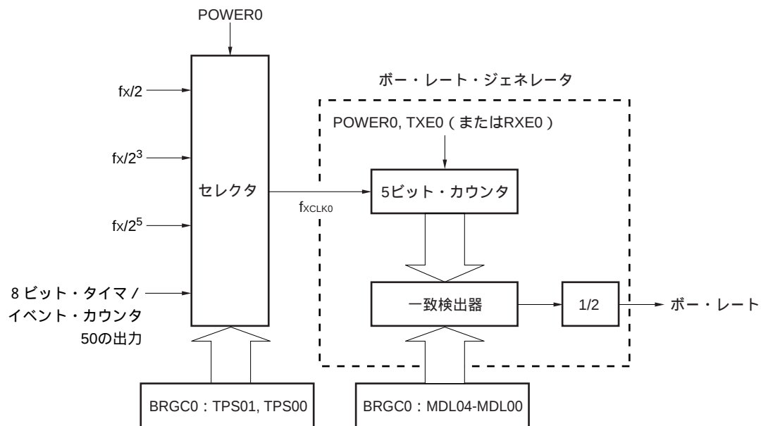
図13 - 11 ポー・レート・ジェネレータの構成
