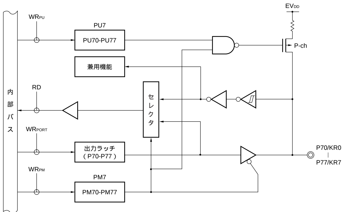
図4 - 17 P70-P77のブロック図
