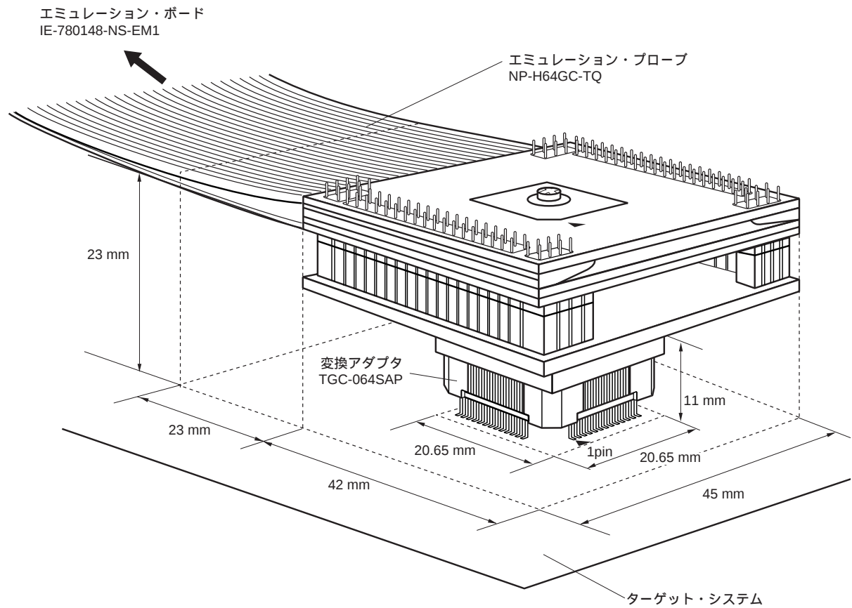
図B - 5 ターゲット・システムの接続条件 (NP-H64GC-TQの場合)
