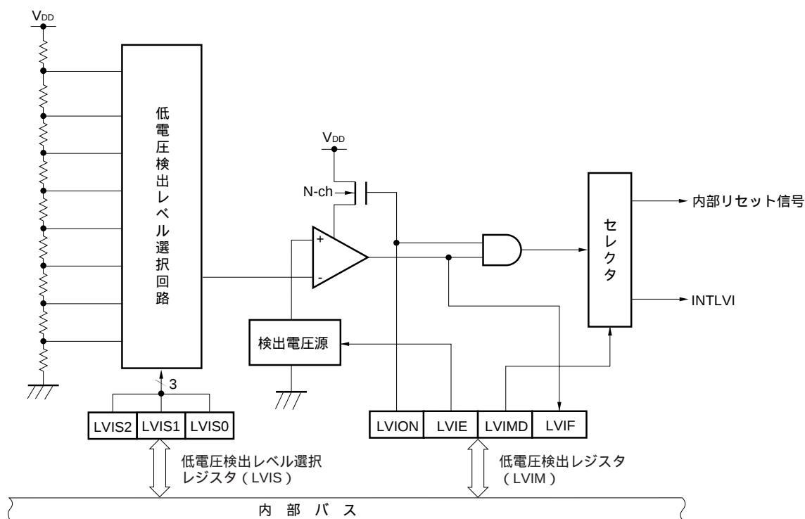
図23 - 1 低電圧検出回路のブロック図
