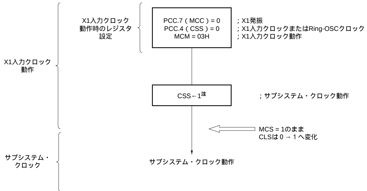
図5 - 16 X1入力クロックからサブシステム・クロックへの切り替え（フロー・チャート）
