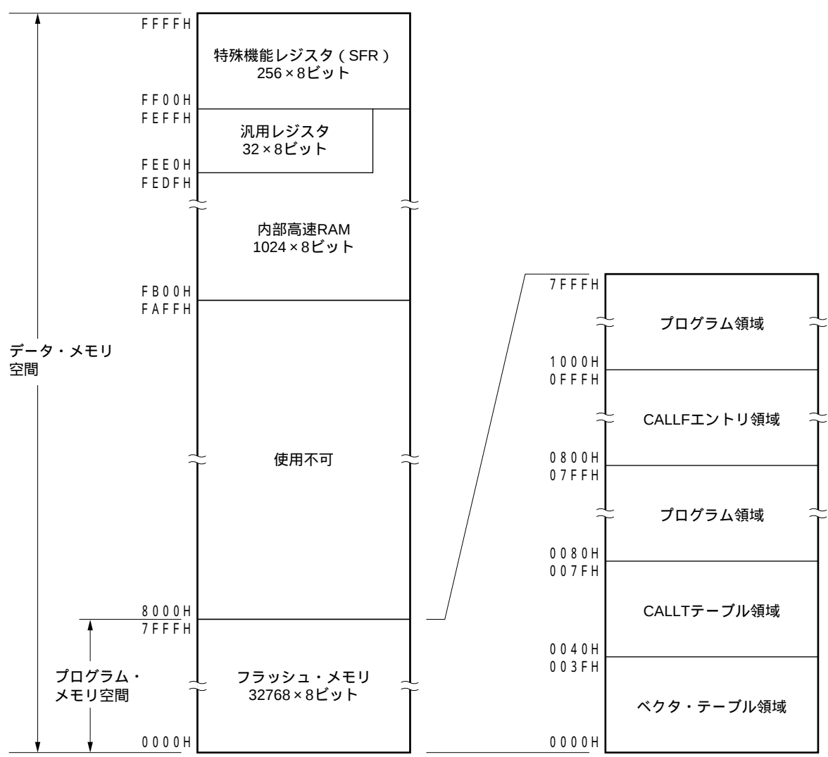
図3 - 5 メモリ・マップ (μ PD78F0134)
