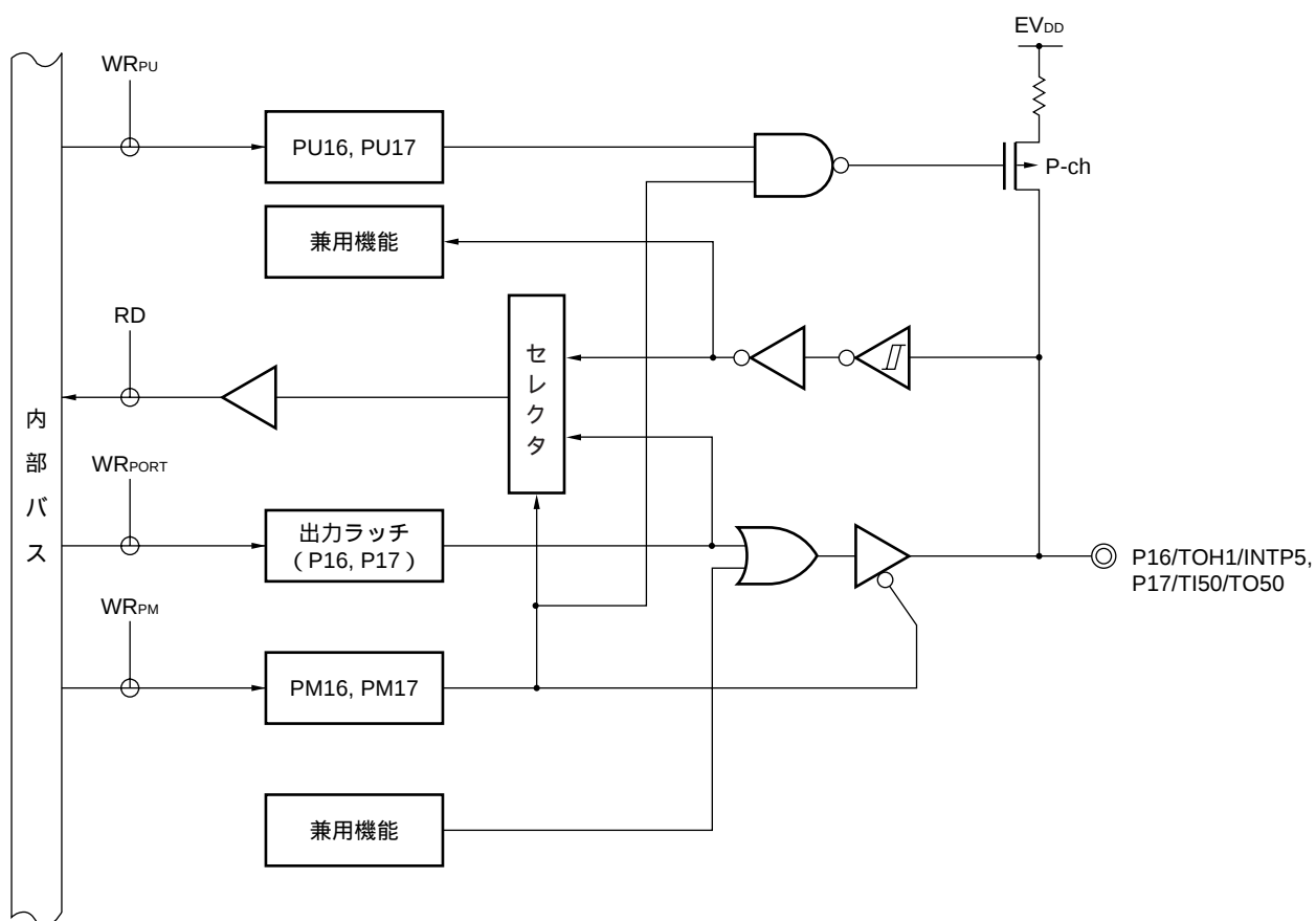
図4 - 10 P16, P17のブロック図
