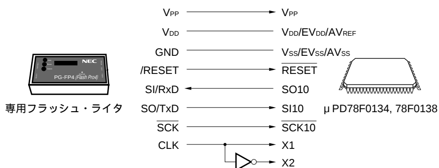
図27 - 9 専用フラッシュ・ライターとの通信 (CSI10)
