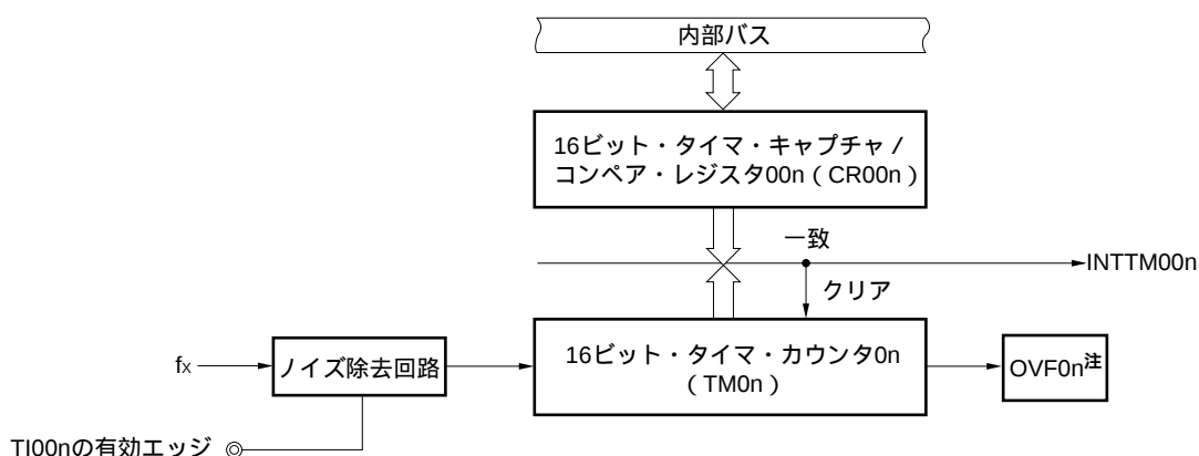
図6 - 32 外部イベント・カウンタの構成図
