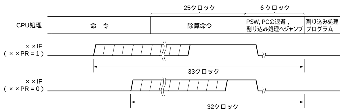
図17 - 9 割り込み要求の受け付けタイミング (最大時間)
