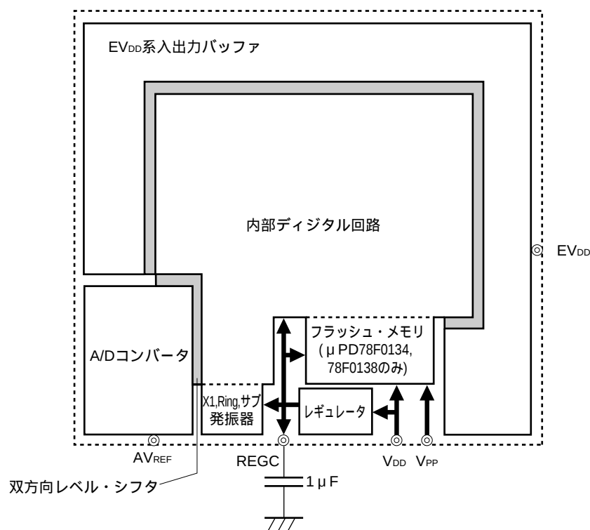
図24 - 1 レギュレータ周辺のブロック図
