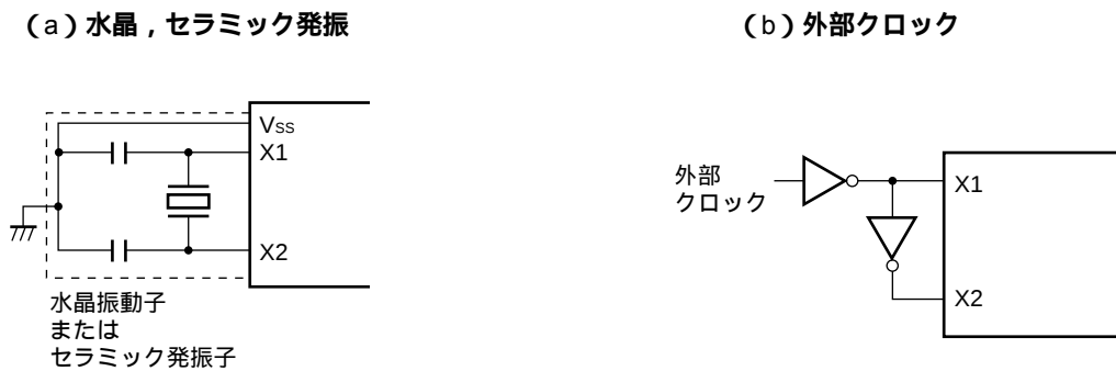
図5 - 8 X1発振回路の外付け回路例
