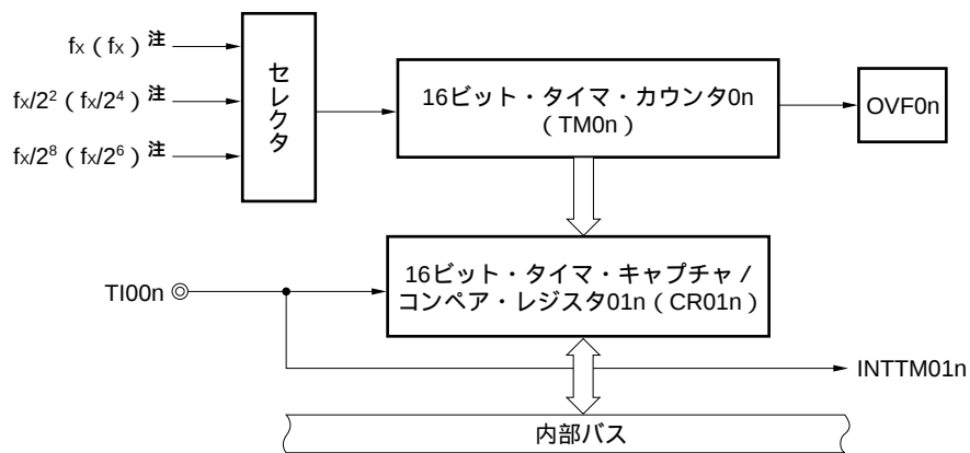
図6 - 23 フリー・ランニング・カウンタによるパルス幅測定の構成図
