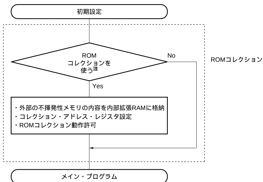
図26 - 6 初期設定ルーチン
