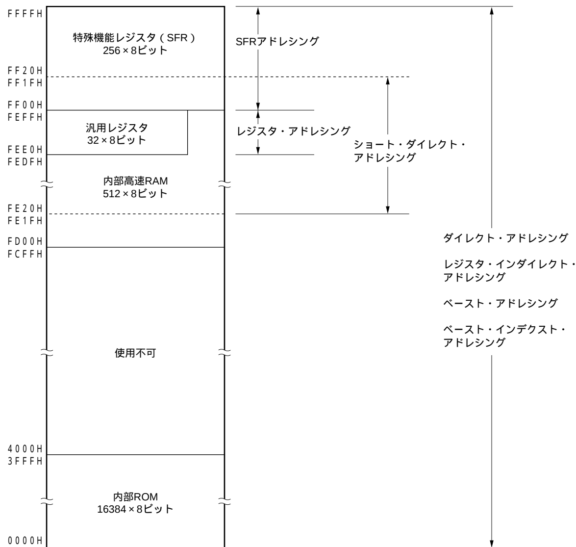
図3 - 10 データ・メモリとアドレッシングの対応 (μPD780132)
