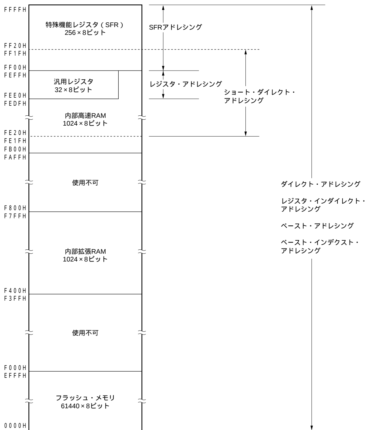
図3 - 16 データ・メモリとアドレッシングの対応 (μ PD78F0138)
