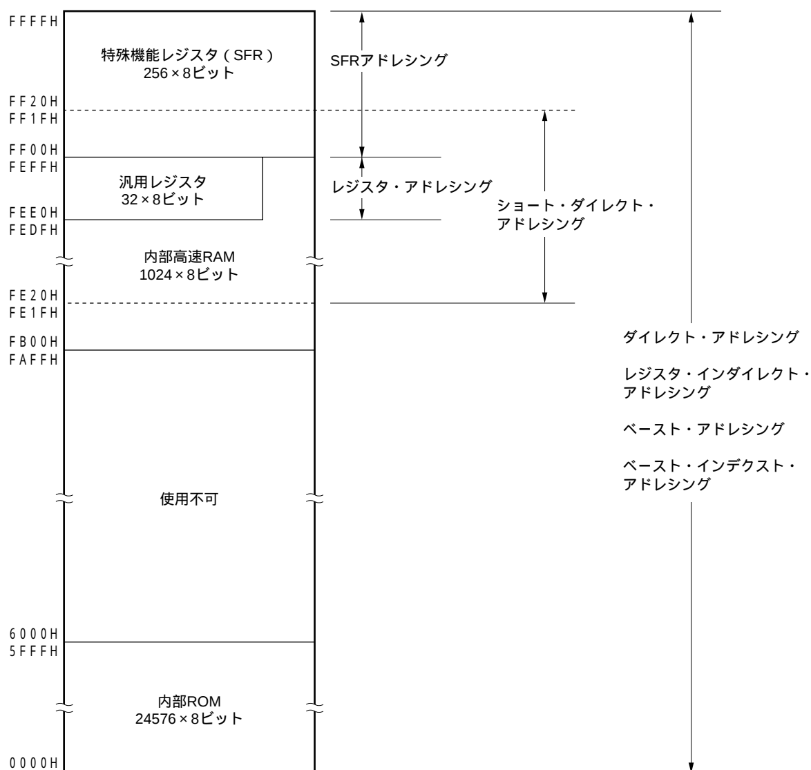
図3 - 11 データ・メモリとアドレッシングの対応 (μPD780133)
