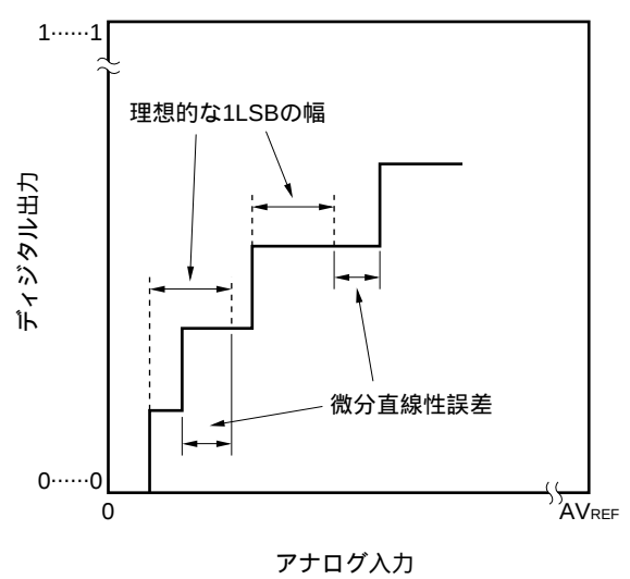
図12 - 18 微分直線性誤差
