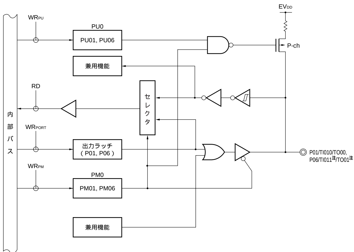
図4 - 3 P01, P06のブロック図
