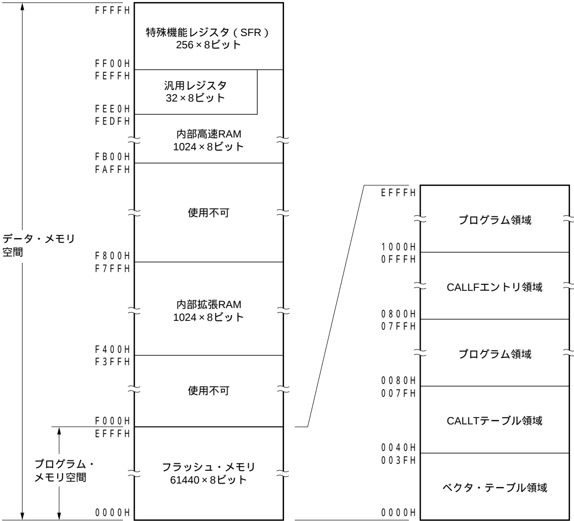
図3 - 8 メモリ・マップ (μ PD78F0138)
