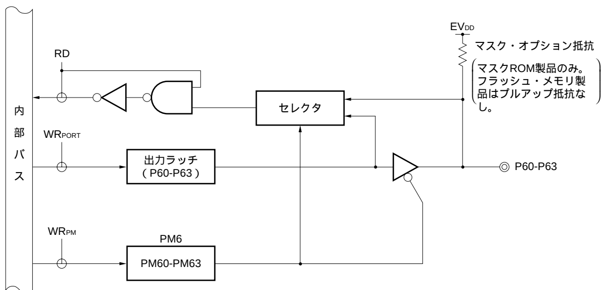
図4 - 16 P60-P63のブロック図
