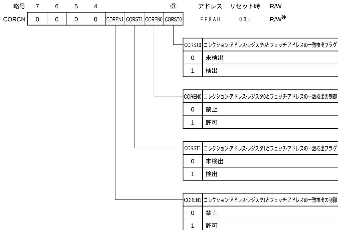
図26-3 コレクション・コントロール・レジスタのフォーマット
