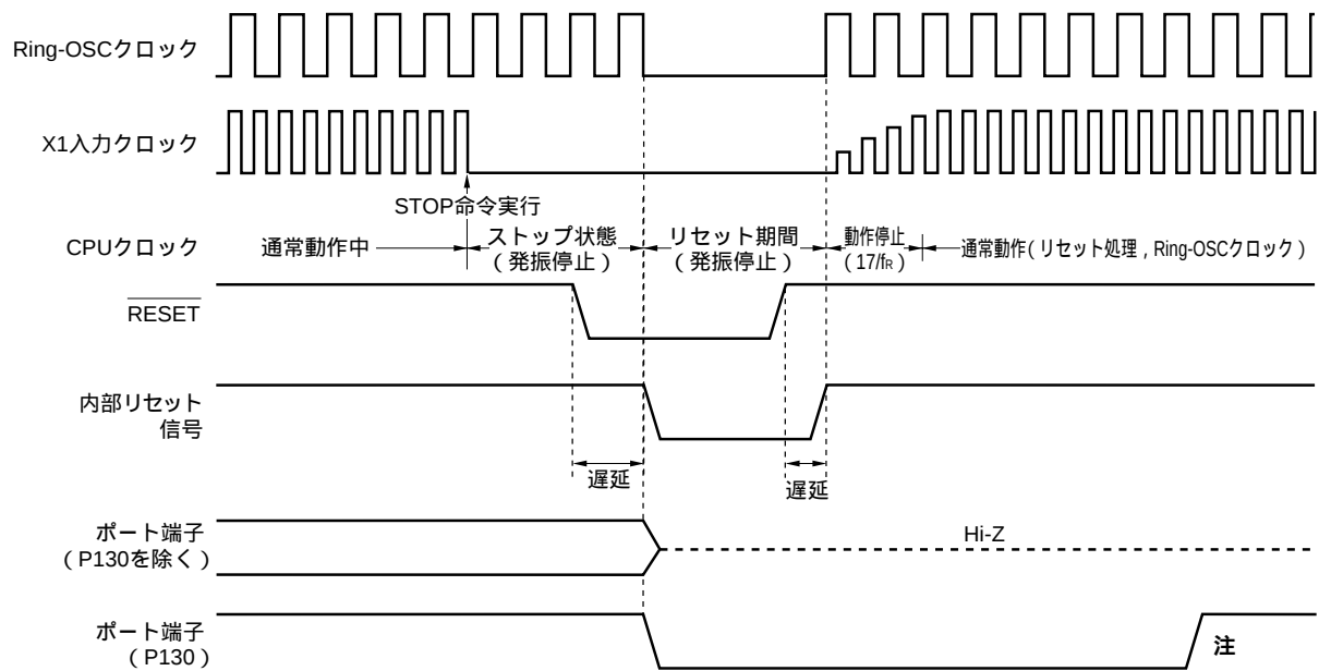
図20 - 4 STOPモード中のRESET入力によるリセット・タイミング
