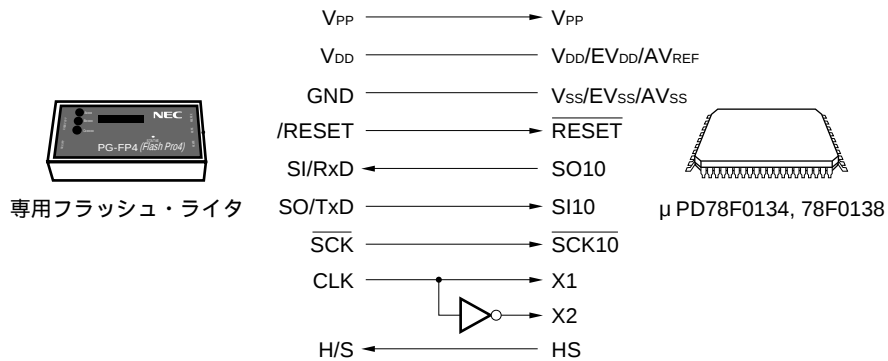
図27 - 10 専用フラッシュ・ライタとの通信 (CSI10 + HS)
