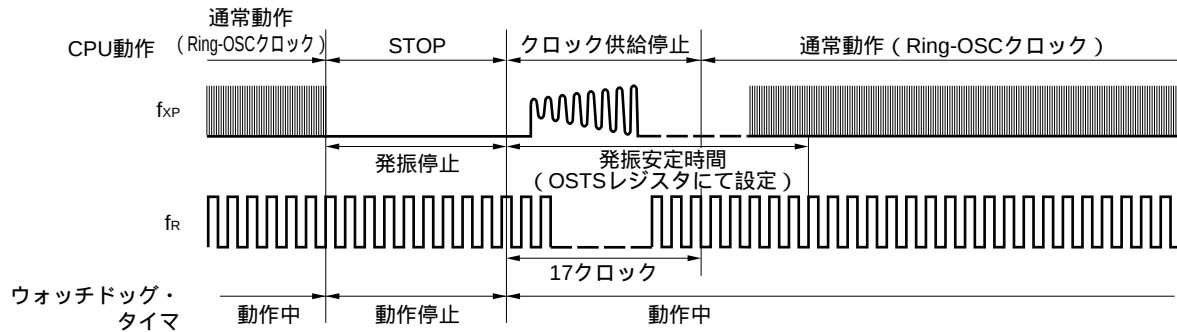
図10 - 7 STOPモード時の動作 (CPUクロックとWDT動作クロック: Ring-OSCクロック)
