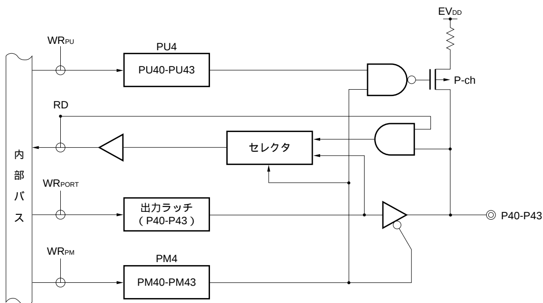
図4 - 14 P40-P43のブロック図
