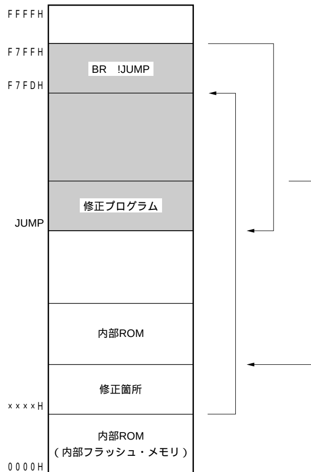
図26 - 8 プログラム遷移図（修正箇所が1つの場合）
