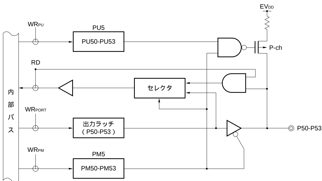
図4 - 15 P50-P53のブロック図
