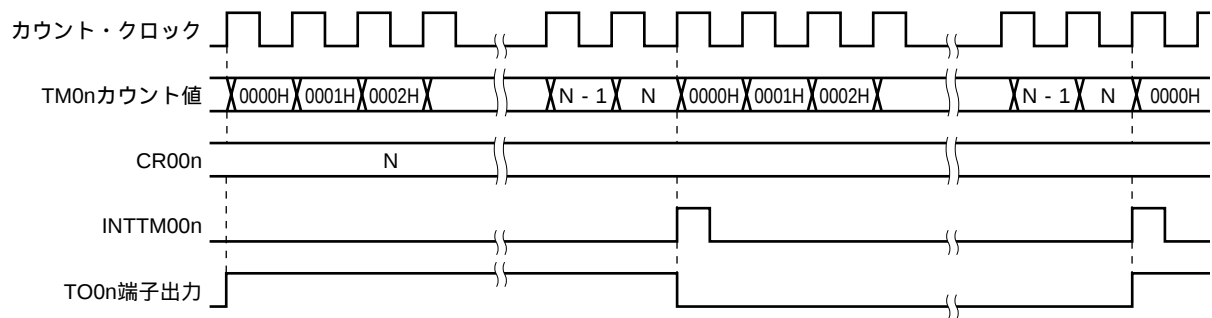
図6 - 35 方形波出力動作のタイミング
