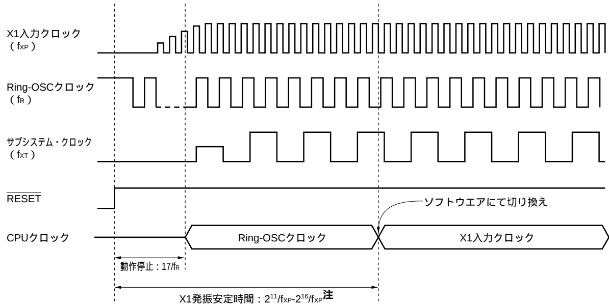
図5 - 12 Ring-OSCによるCPUデフォルト・スタートのタイミング図
