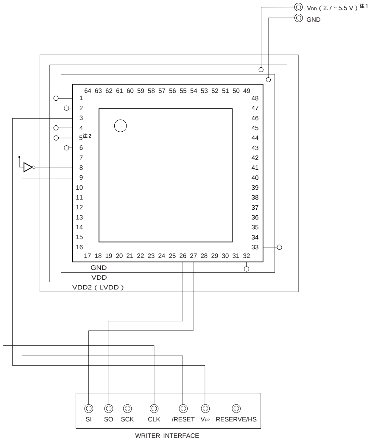
図27 - 5 UART (UART0) 方式でのフラッシュ書き込み用アダプタ配線例
