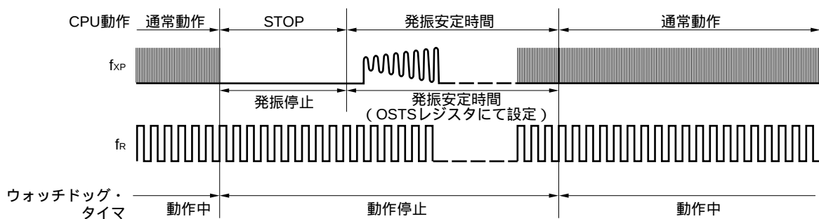
図10 - 4 STOPモード時の動作（CPUクロックとWDT動作クロック：X1入力クロック）
