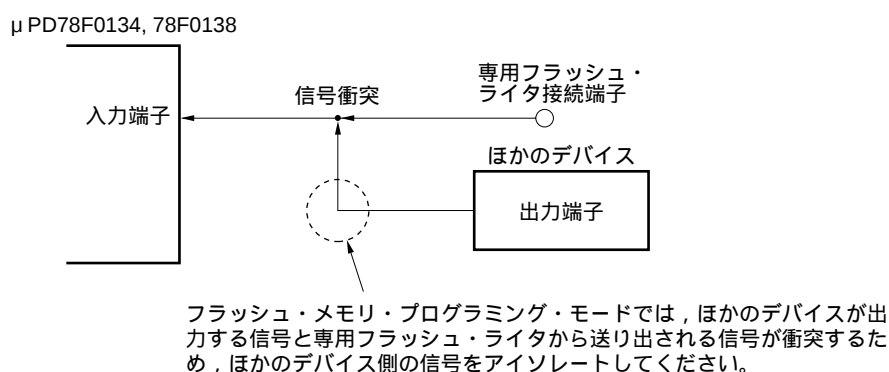
図27 - 15 信号の衝突 (シリアル・インタフェースの入力端子)
