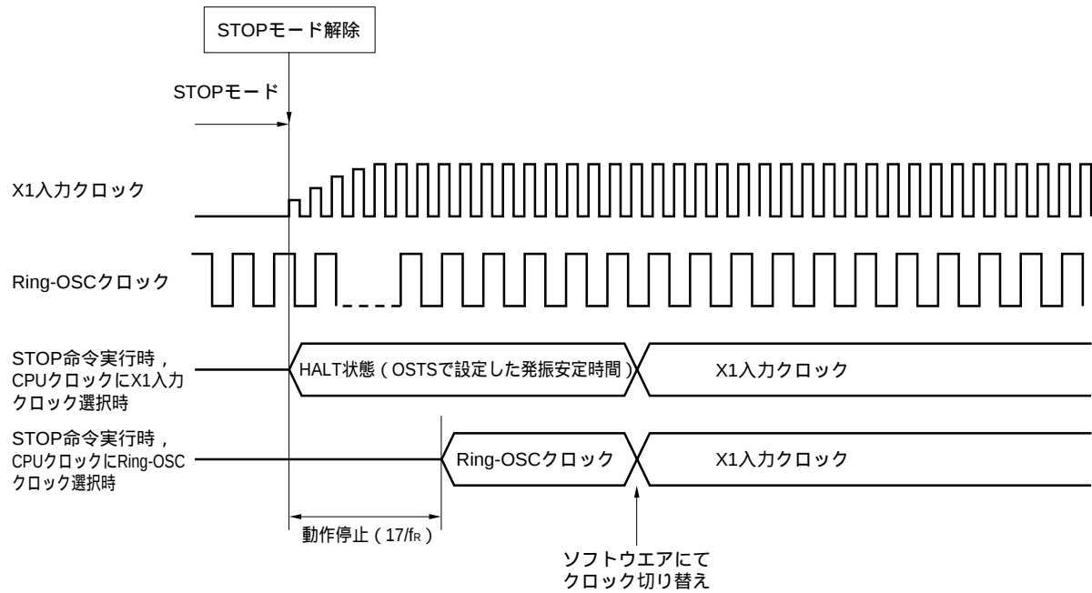
図19 - 5 STOPモード解除時の動作タイミング
