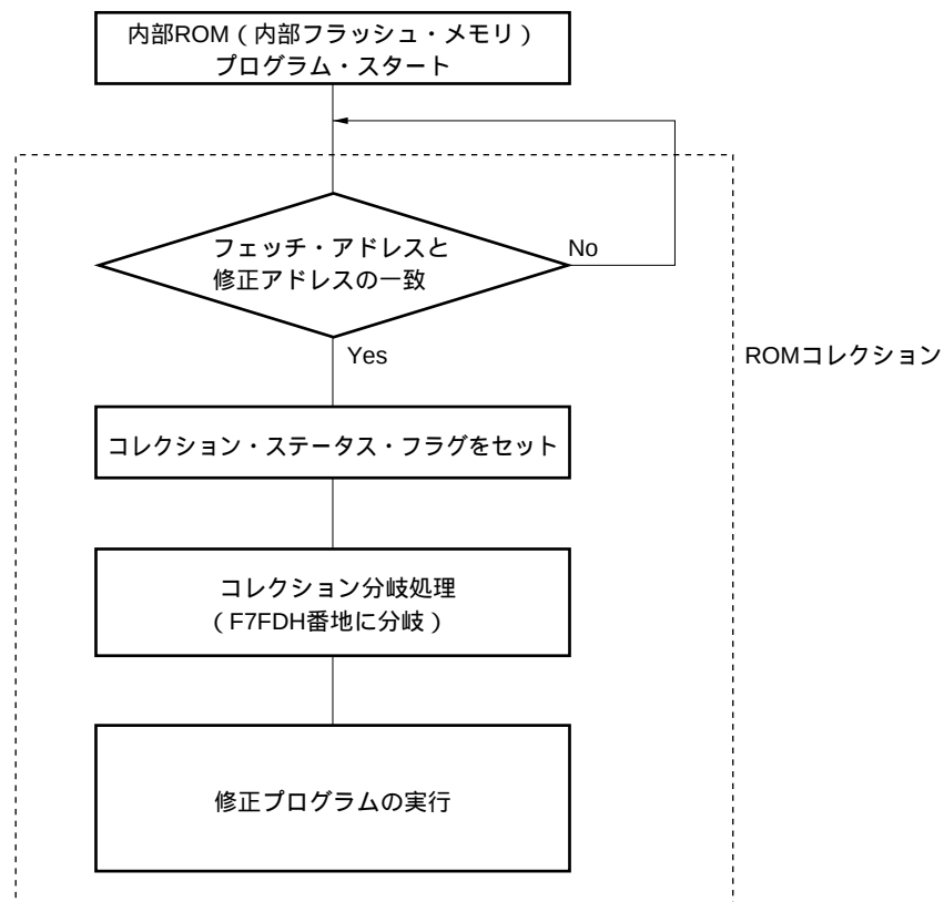
図26 - 7 ROMコレクションの動作
