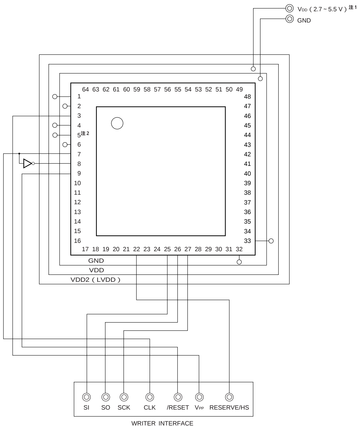
図27 - 4 3線式シリアルI/O (CSI10+HS)方式でのフラッシュ書き込み用アダプタ配線例
