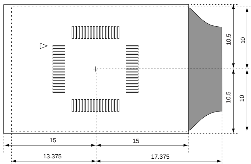
図B - 8 ターゲット・システム上の制限領域 (64ピンGBパッケージの場合)
