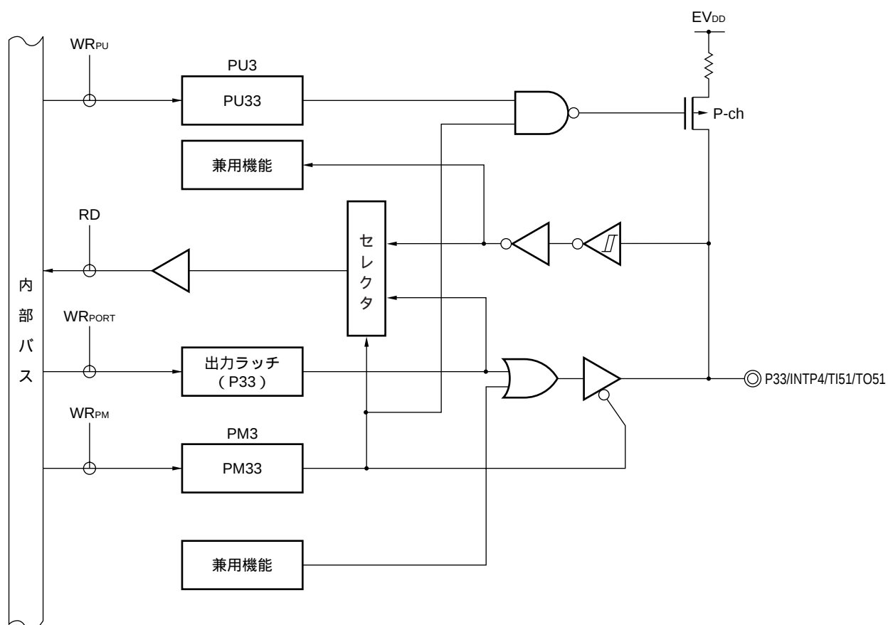
図4 - 13 P33のブロック図
