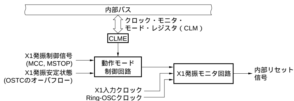
図21 - 1 クロック・モニタのブロック図
