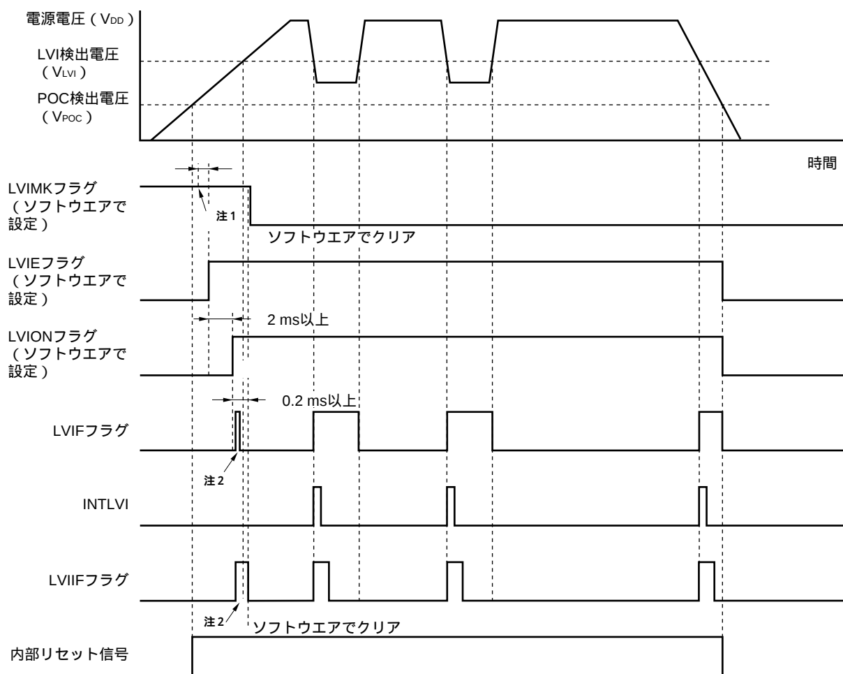
図23 - 5 低電圧検出回路の割り込み信号発生タイミング
