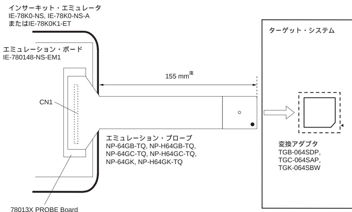
図B - 1 IEシステムから変換アダプタまでの距離
