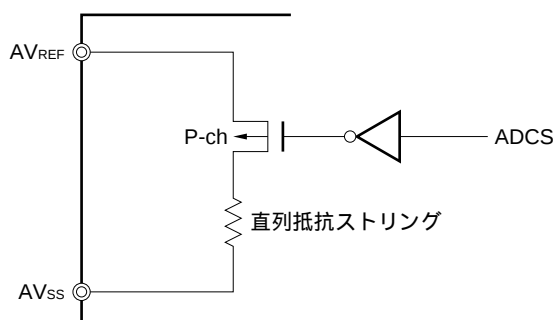
図12 - 2 直列抵抗ストリングの回路構成
