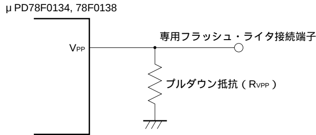
図27 - 14 V PP 端子の接続例
