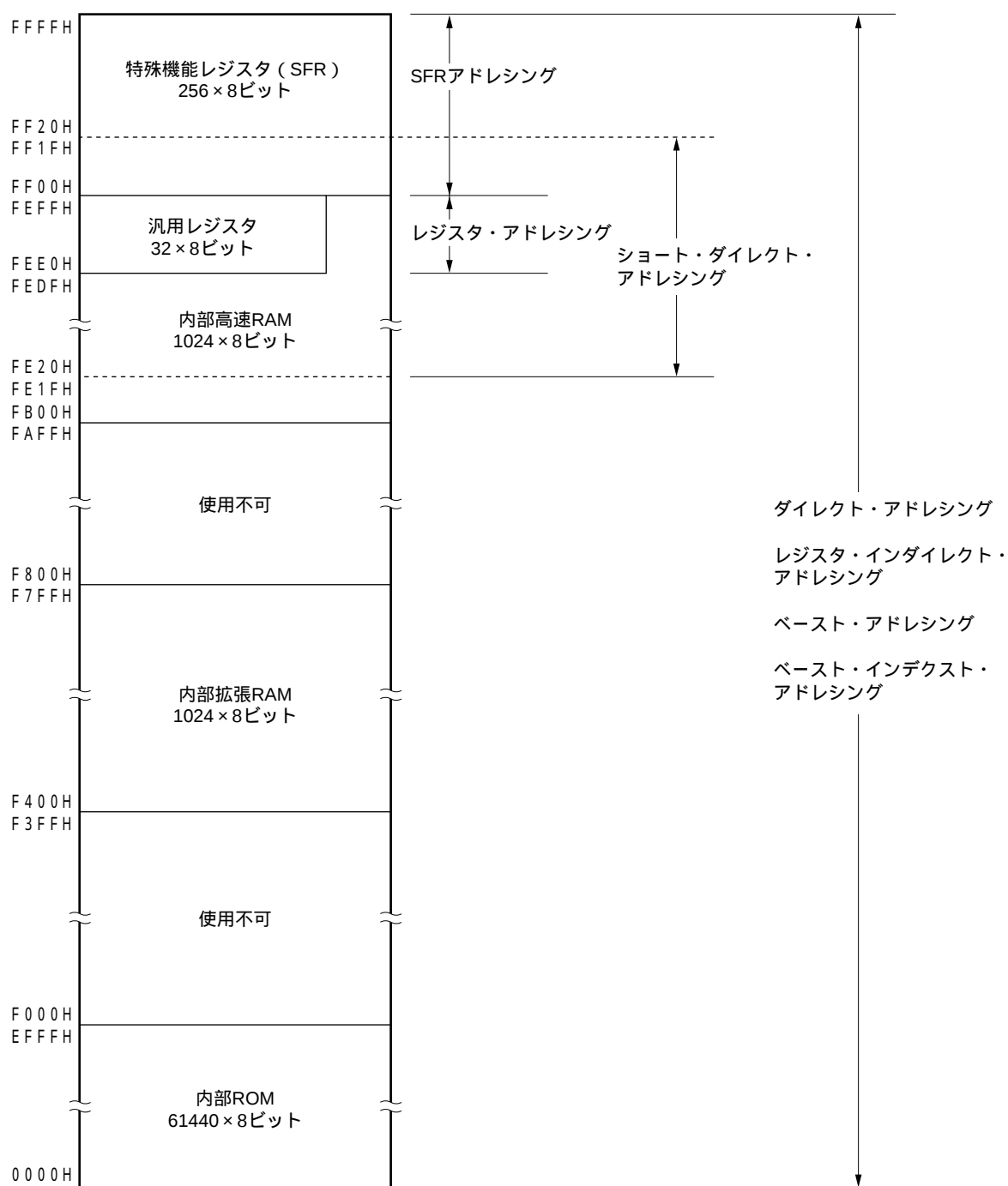
図3 - 15 データ・メモリとアドレッシングの対応 (μ PD780138)
