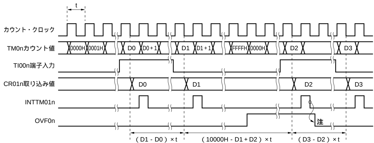
図6 - 24 フリー・ランニング・カウンタとキャプチャ・レジスタ1本によるパルス幅測定動作のタイミング (両エッジ指定時)
