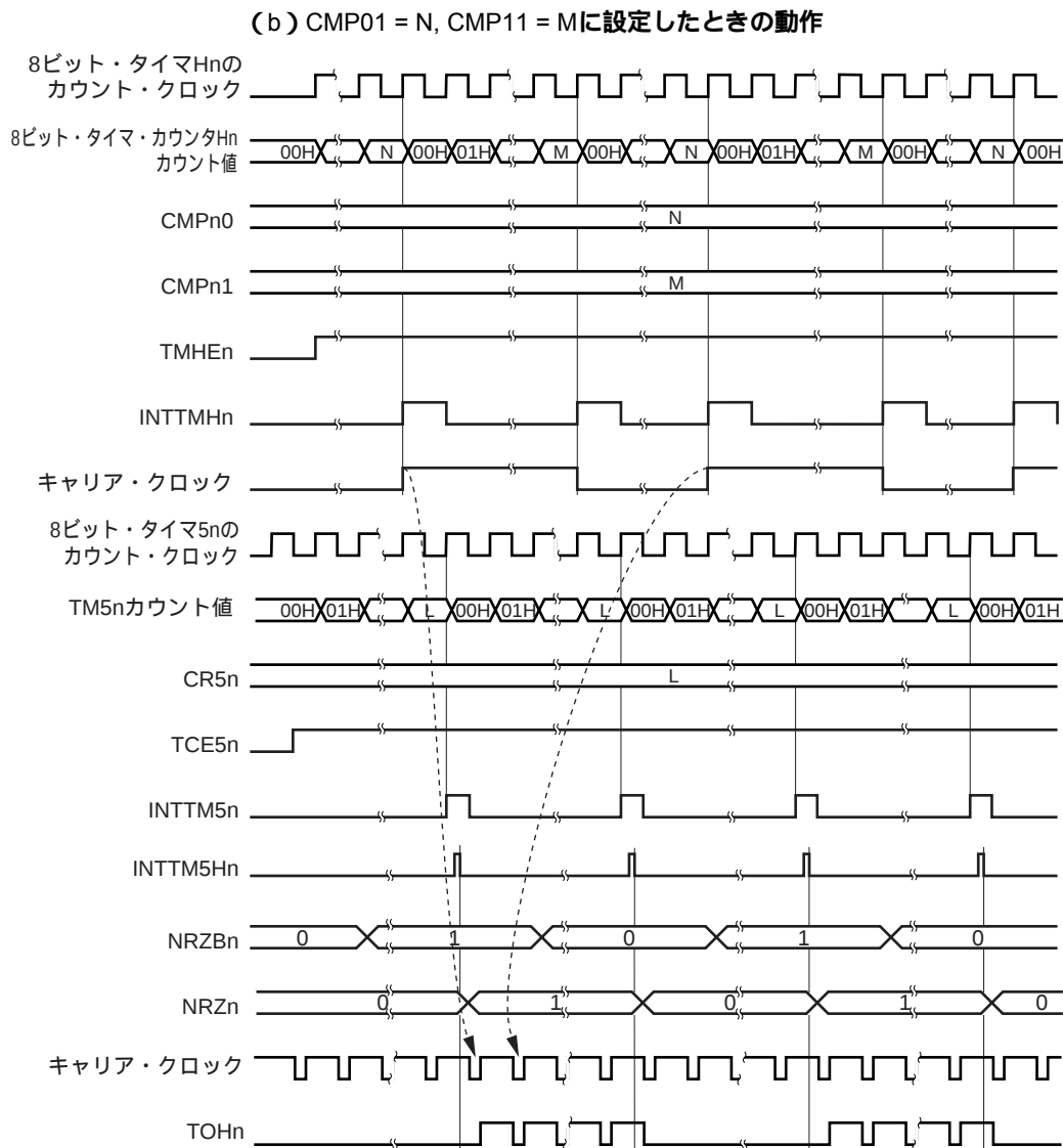
図8 - 15 キャリア・ジェネレータ・モード動作のタイミング (2/3)
