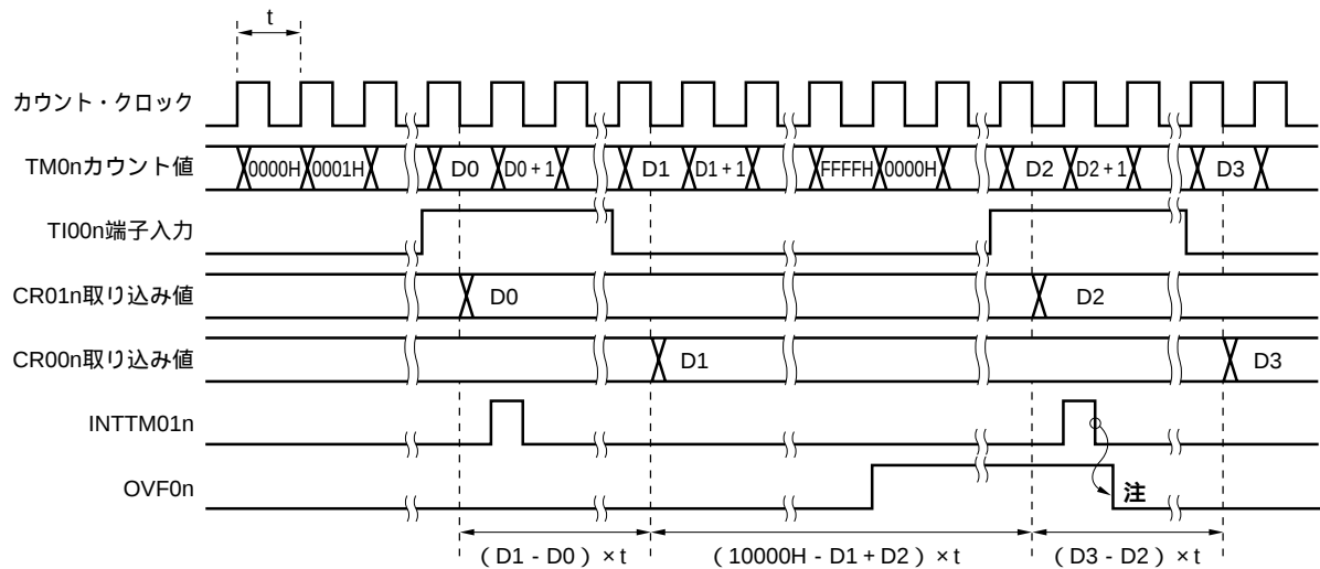
図6 - 28 フリー・ランニング・カウンタとキャプチャ・レジスタ2本によるパルス幅測定動作のタイミング (立ち上がりエッジ指定時)
