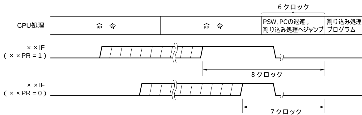
図17 - 8 割り込み要求の受け付けタイミング (最小時間)
