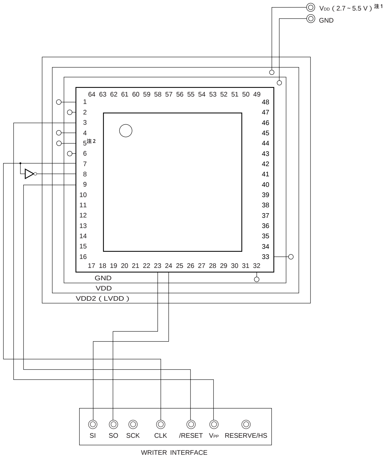
図27 - 7 UART (UART6) 方式でのフラッシュ書き込み用アダプタ配線例
