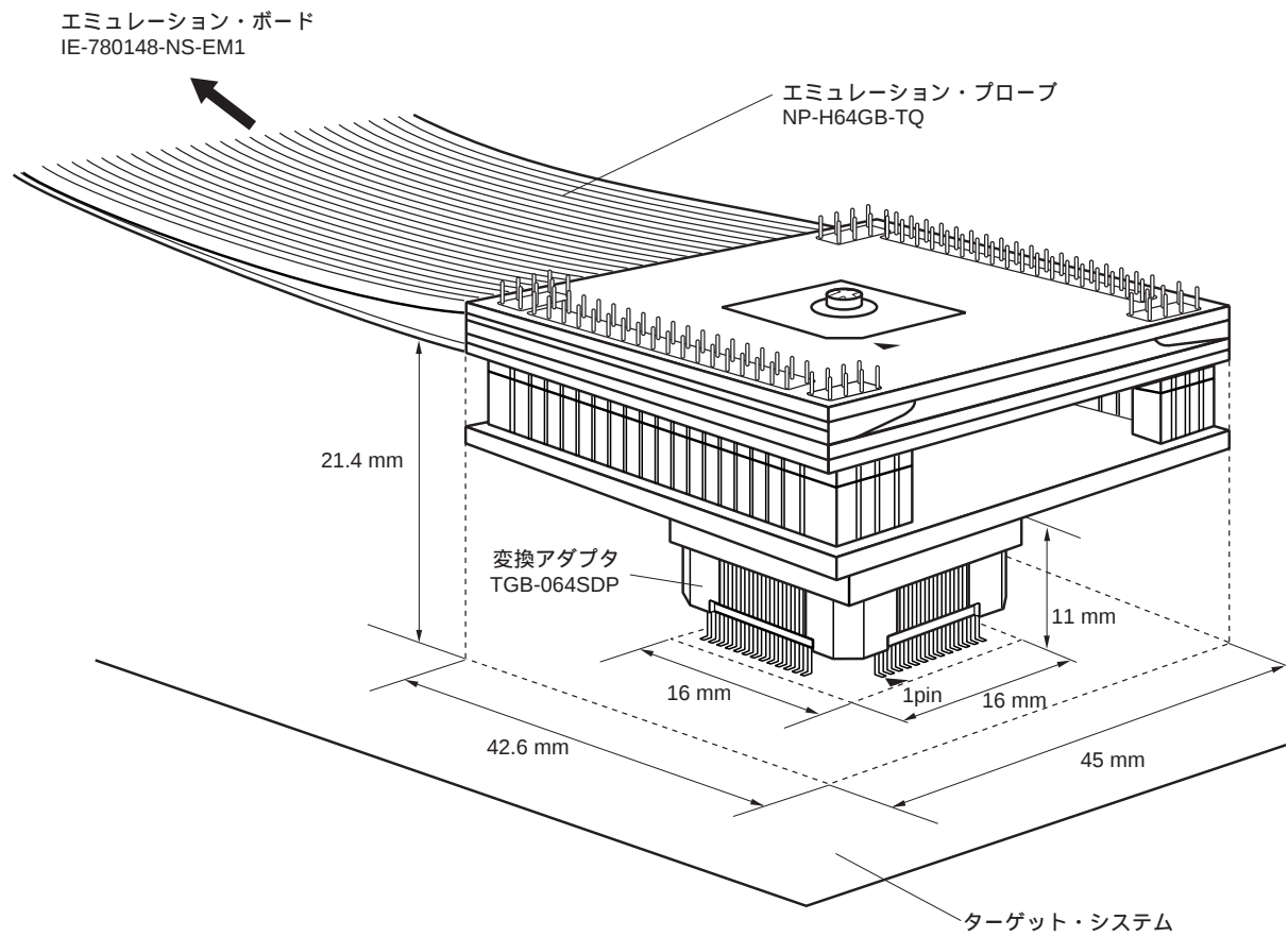
図B - 3 ターゲット・システムの接続条件 (NP-H64GB-TQの場合)
