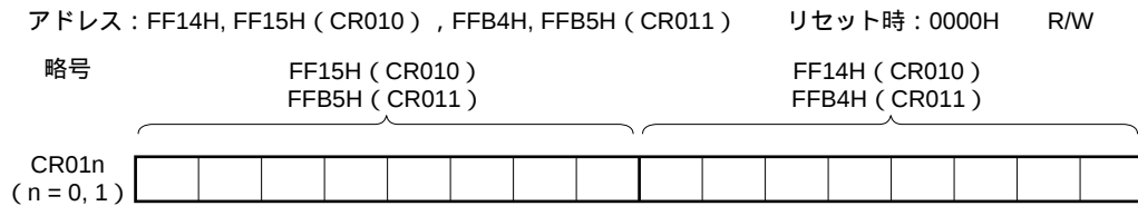
図6 - 5 16ビット・タイマ・キャプチャ/コンペア・レジスタ01n (CR01n) のフォーマット
