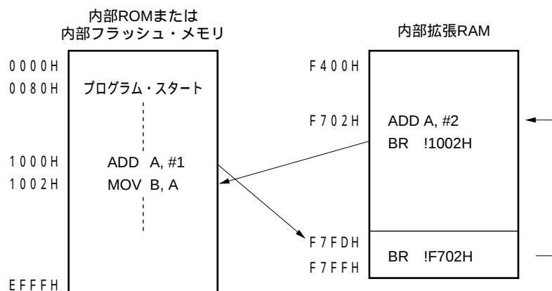
図26 - 4 ROMコレクションの使用例
