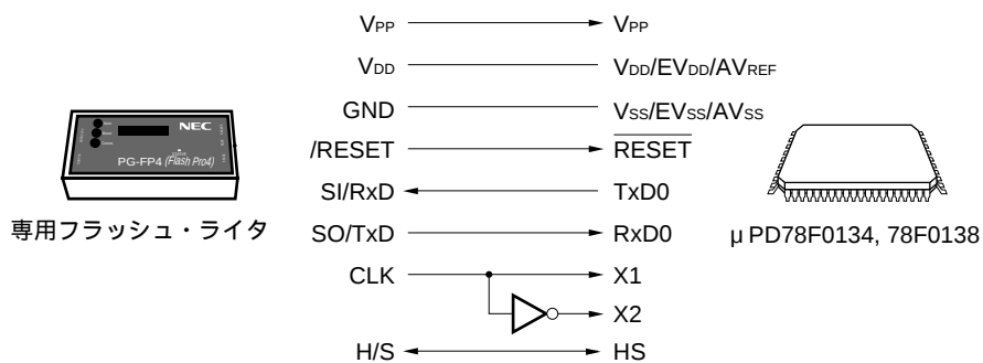
図27 - 12 専用フラッシュ・ライタとの通信 (UART0 + HS)
