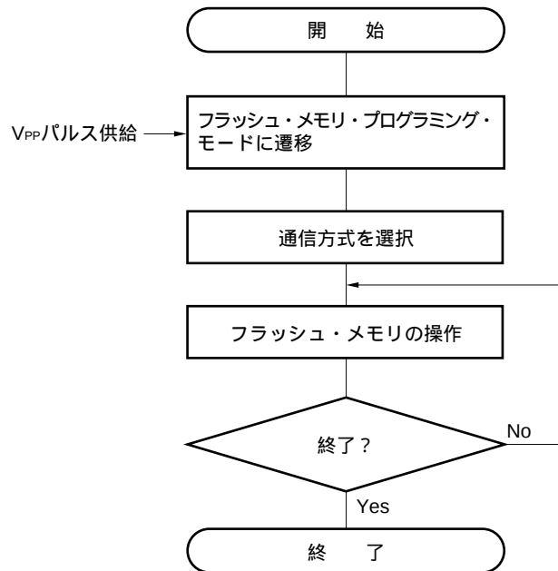
図27 - 18 フラッシュ・メモリの操作手順
