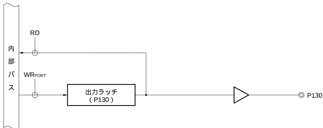
図4 - 19 P130のブロック図
