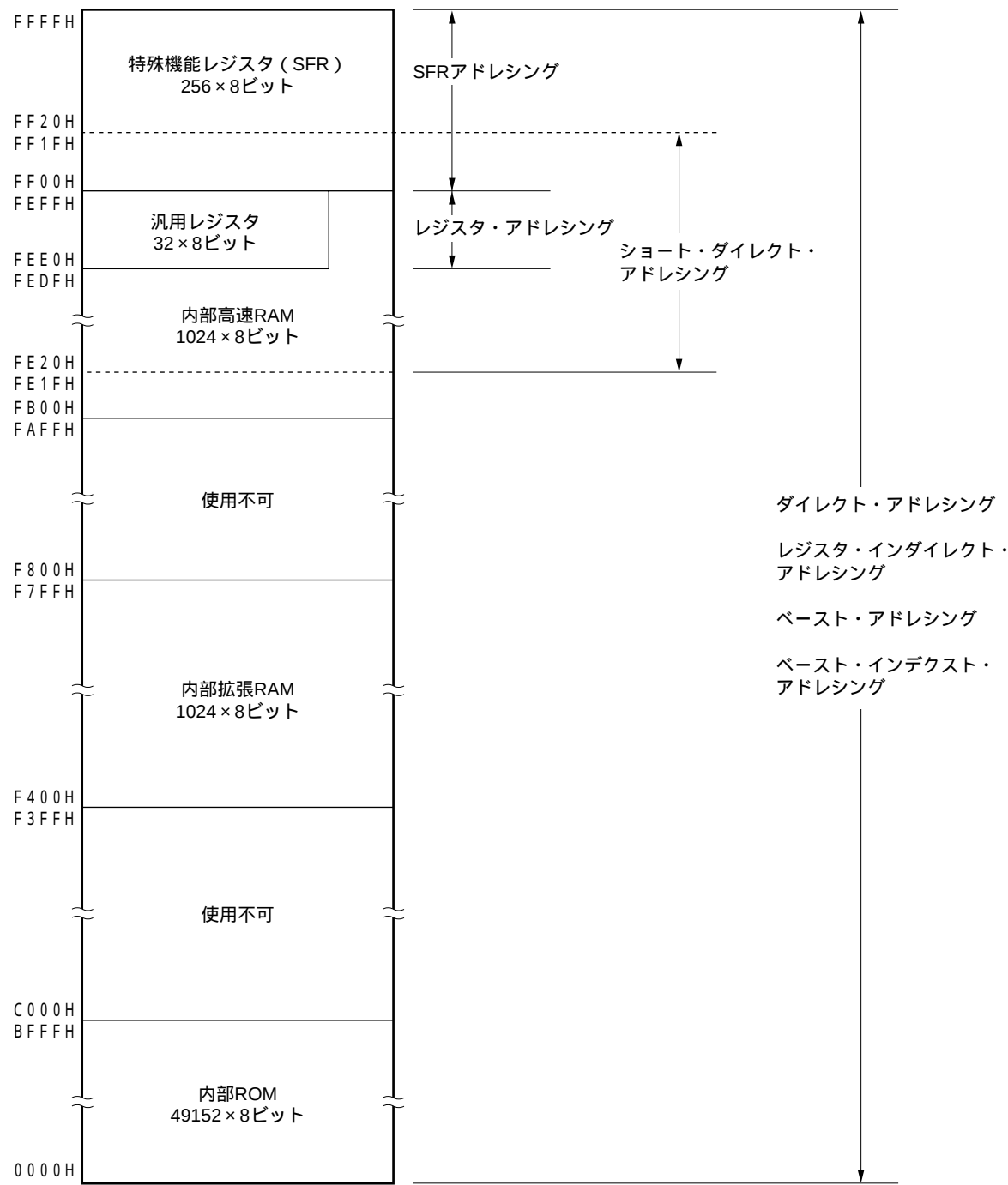
図3 - 14 データ・メモリとアドレッシングの対応 (μ PD780136)
