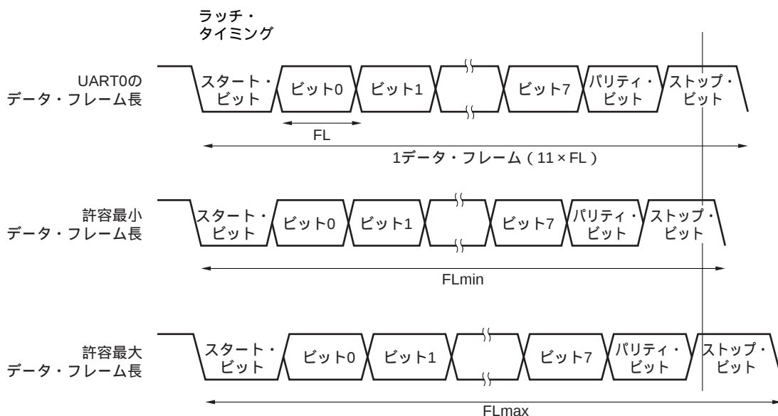
図13-12 受信時の許容ボー・レート範囲
