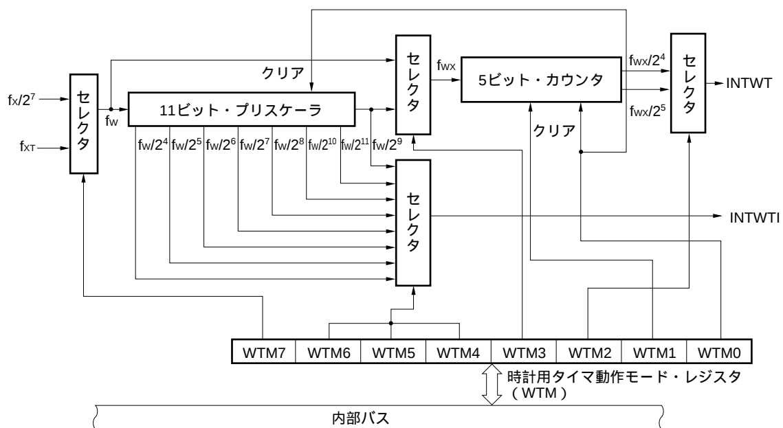
図9 - 1 時計用タイマのブロック図
