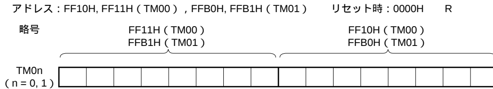
図6 - 3 16ビット・タイマ・カウンタ0n (TM0n) のフォーマット
