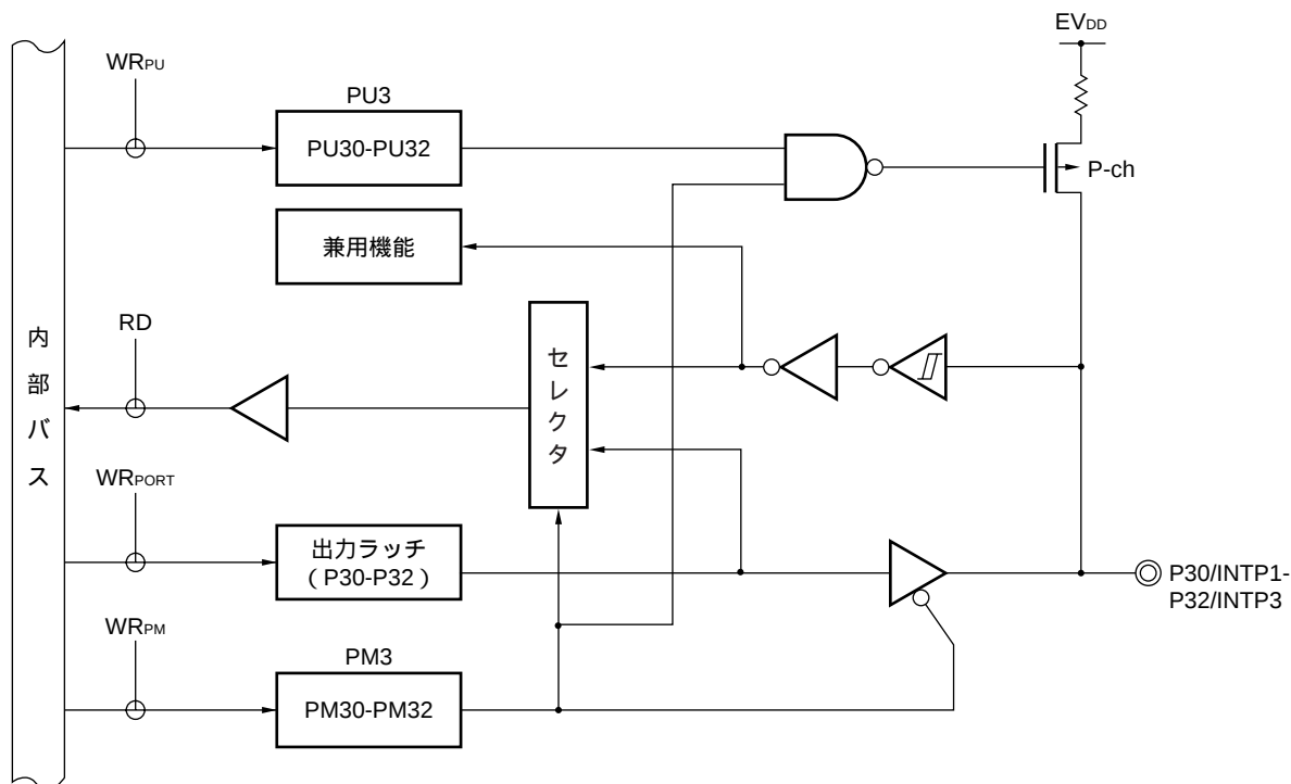
図4 - 12 P30-P32のブロック図
