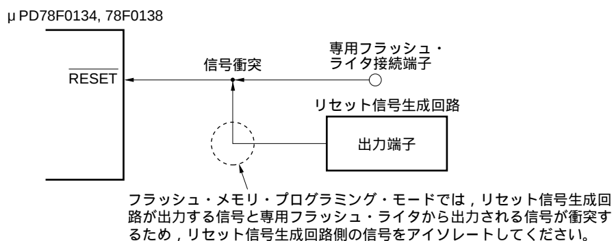
図27 - 17 信号の衝突 ( \overline{\text{RESET}} 端子)
