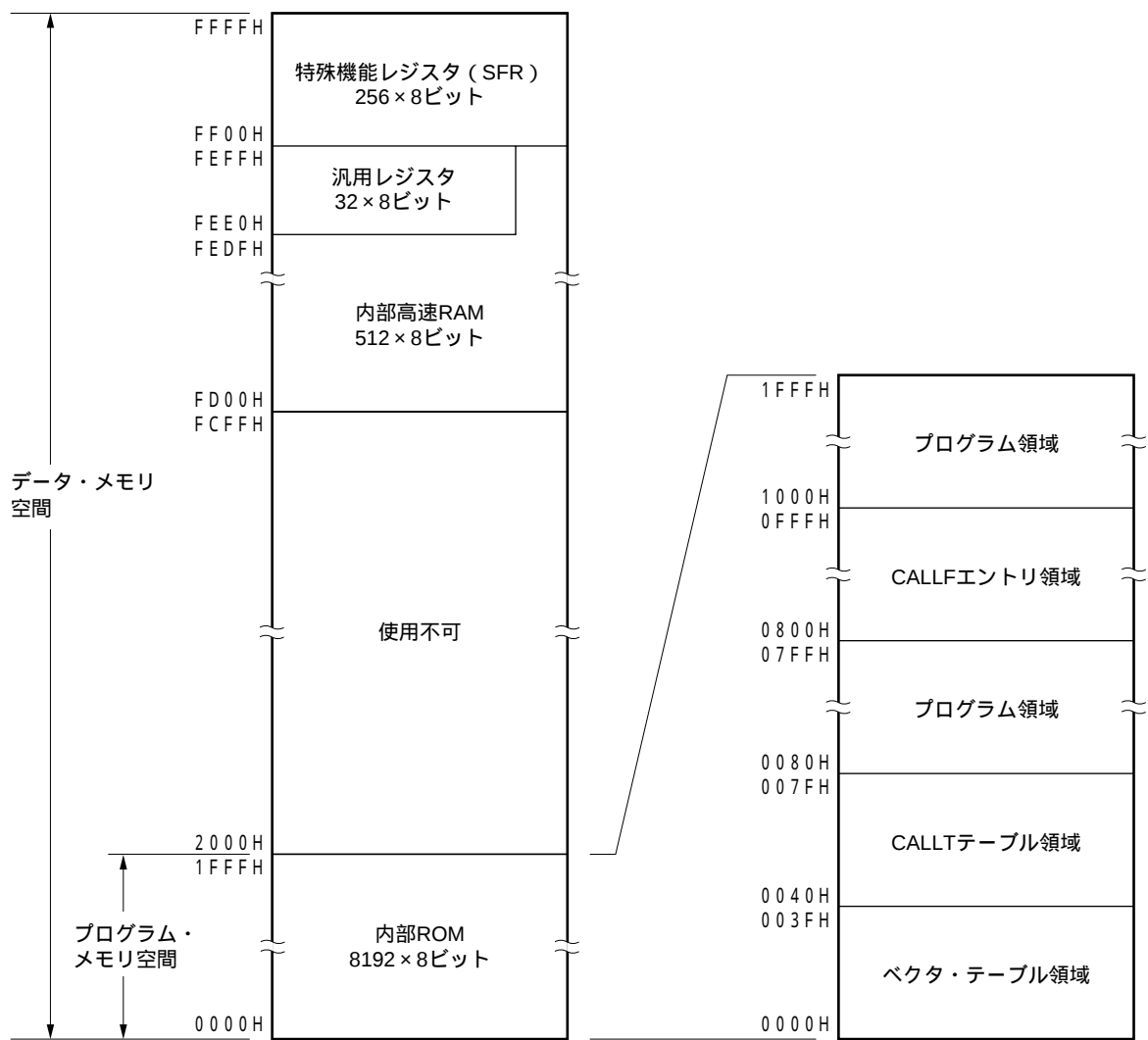
図3 - 1 メモリ・マップ (μPD780131)
