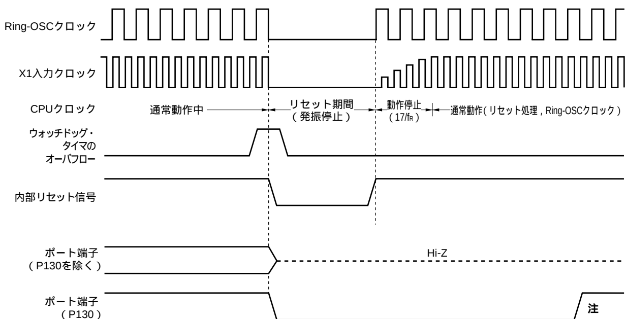
図20 - 3 ウォッチドッグ・タイマのオーバーフローによるリセット・タイミング
