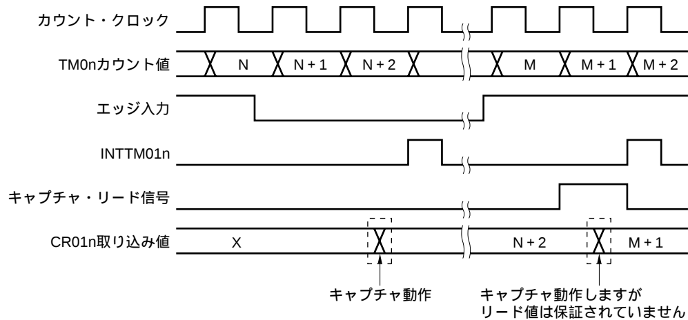
図6 - 42 キャプチャ・レジスタのデータ保持タイミング
