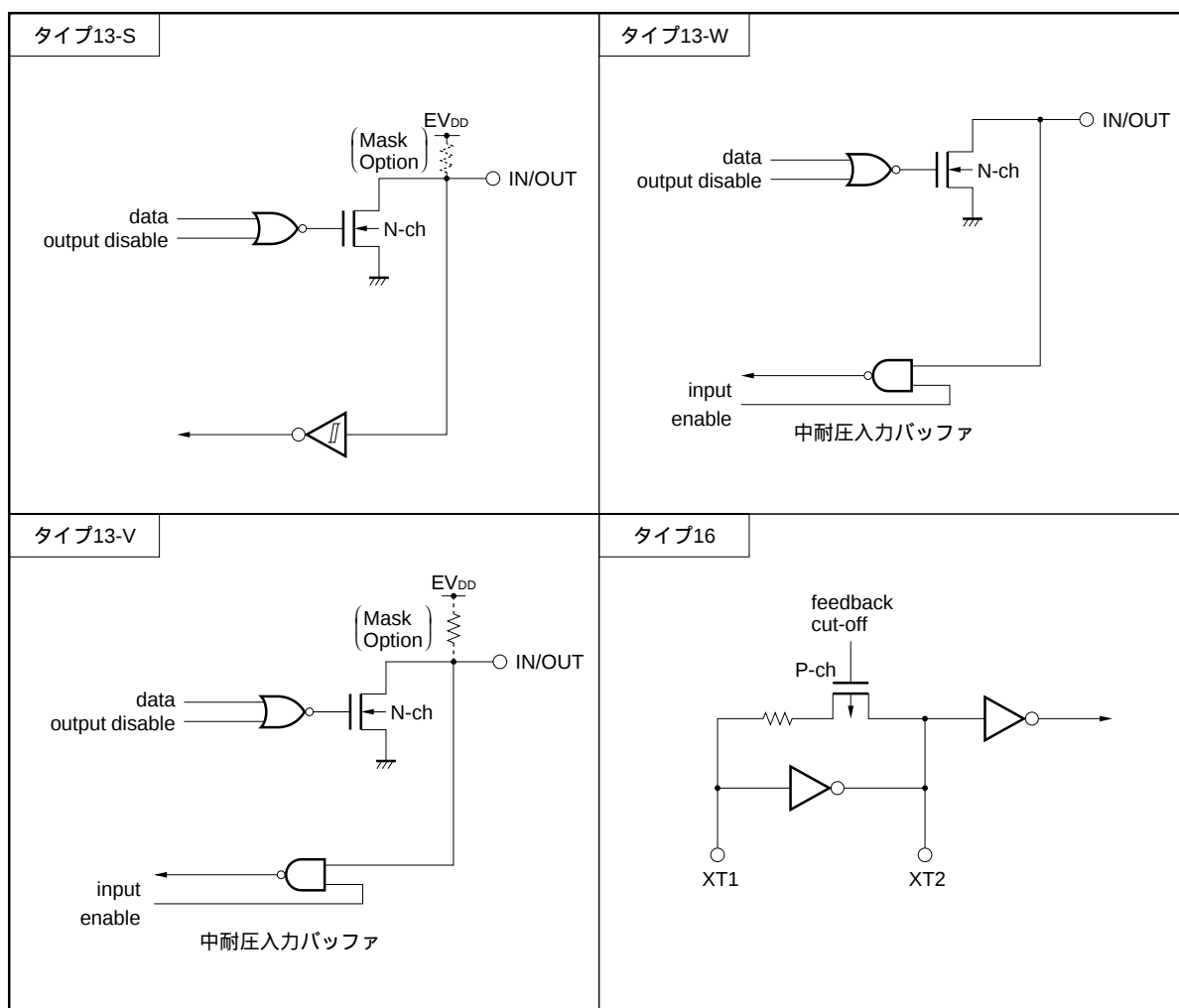
図2 - 1 端子の入出力回路一覧 (2/2)
