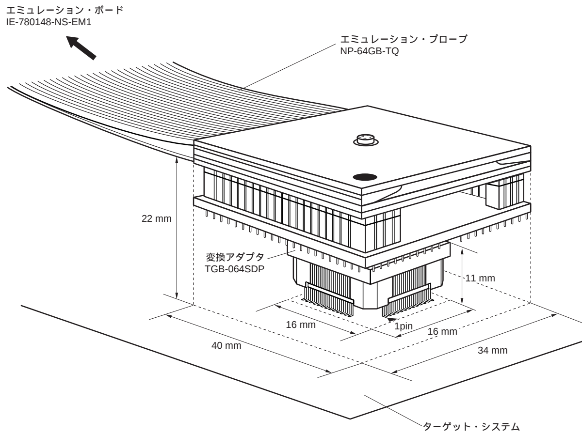
図B - 2 ターゲット・システムの接続条件 (NP-64GB-TQの場合)
