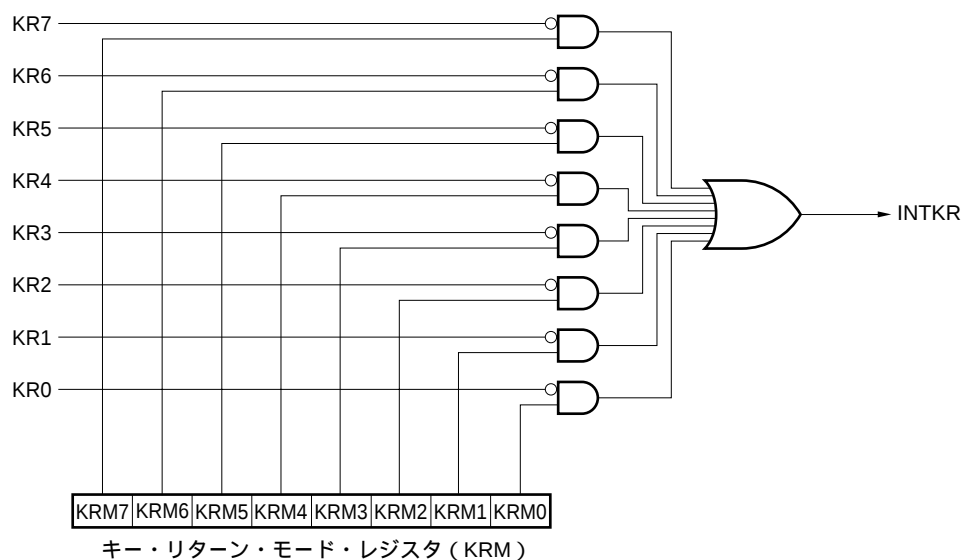
図18 - 1 キー割り込みのブロック図
