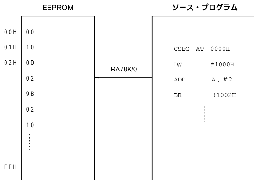
図26 - 5 EEPROMへの格納例（修正箇所が1つの場合）
