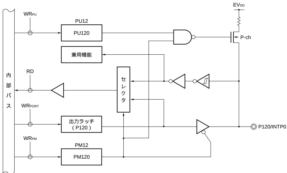
図4 - 18 P120のブロック図
