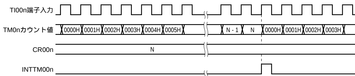
図6 - 33 外部イベント・カウンタ動作のタイミング (立ち上がりエッジ指定時)
