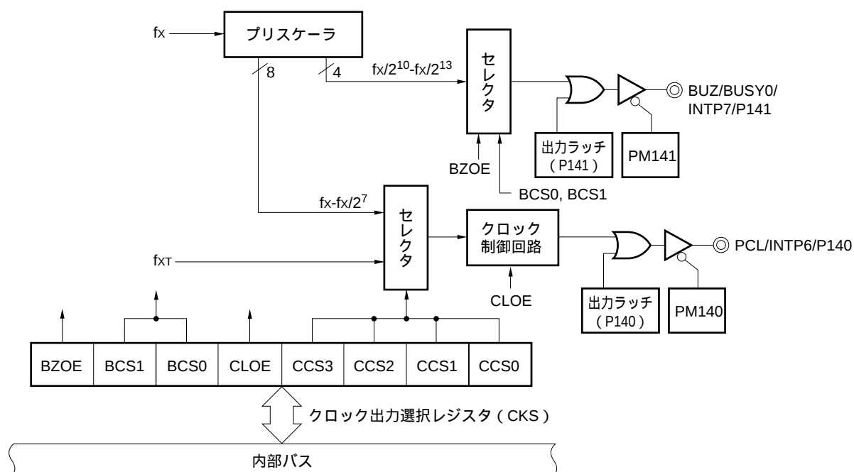
図11 - 1 クロック出力／ブザー出力制御回路のブロック図
