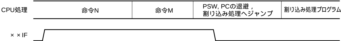
図17 - 11 割り込み要求の保留
