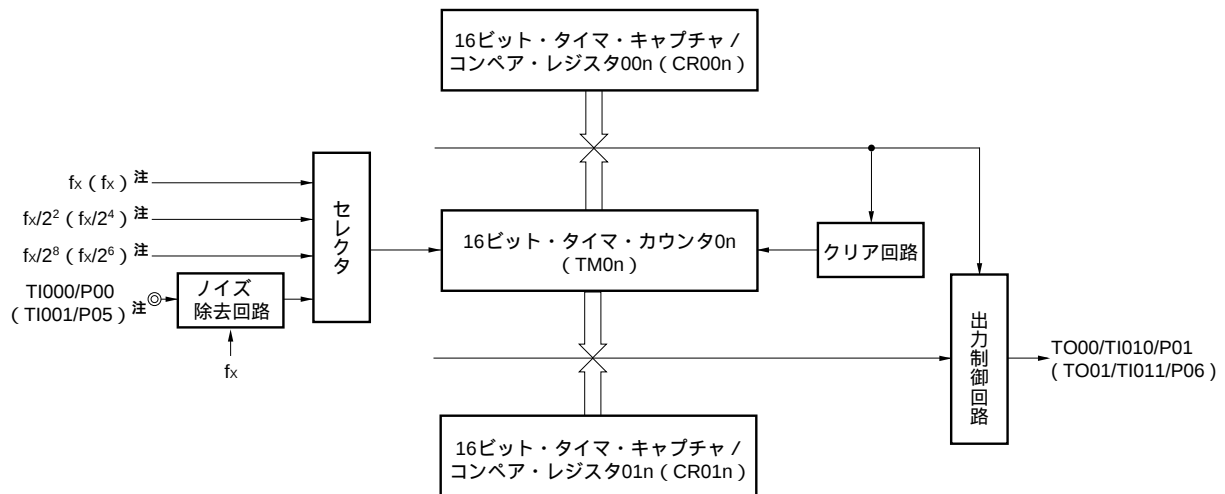
図6 - 19 PPG出力の構成図
