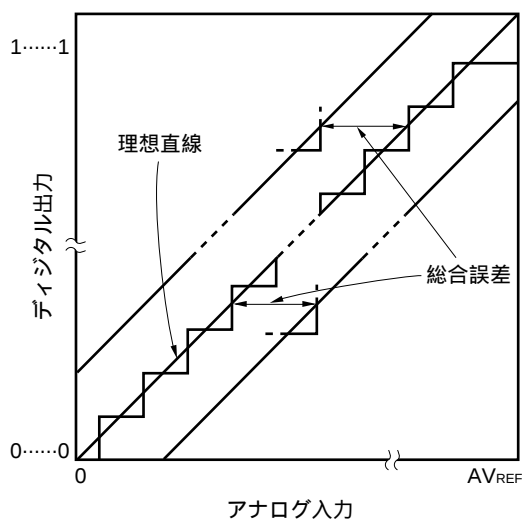
図12 - 13 総合誤差
