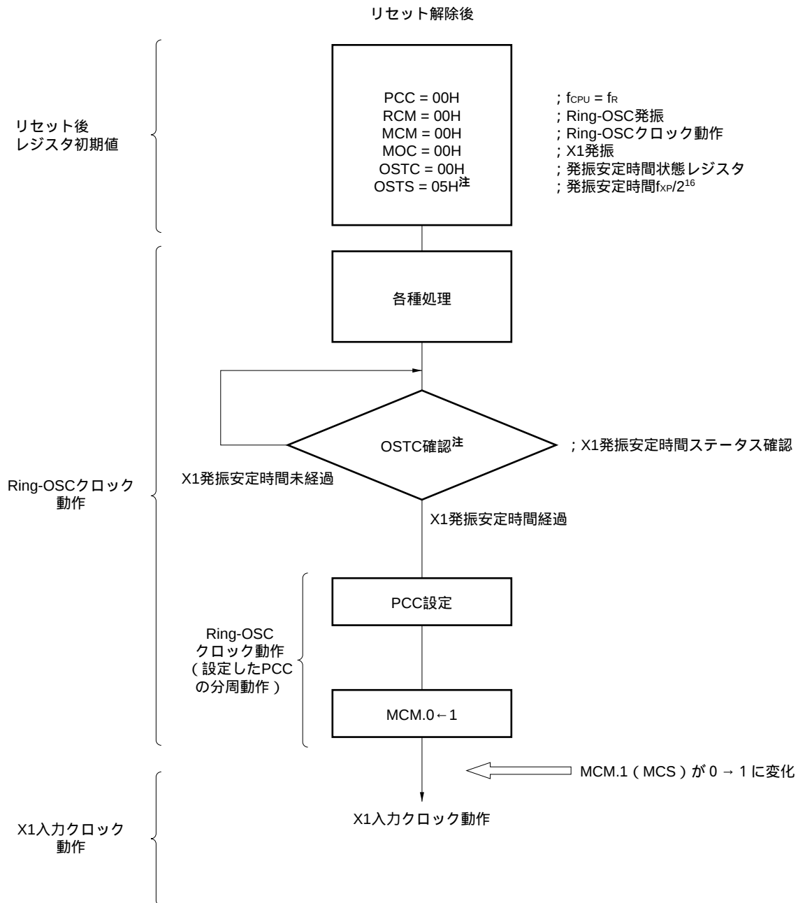
図5 - 14 Ring-OSCクロックからX1入力クロックへの切り替え（フロー・チャート）
