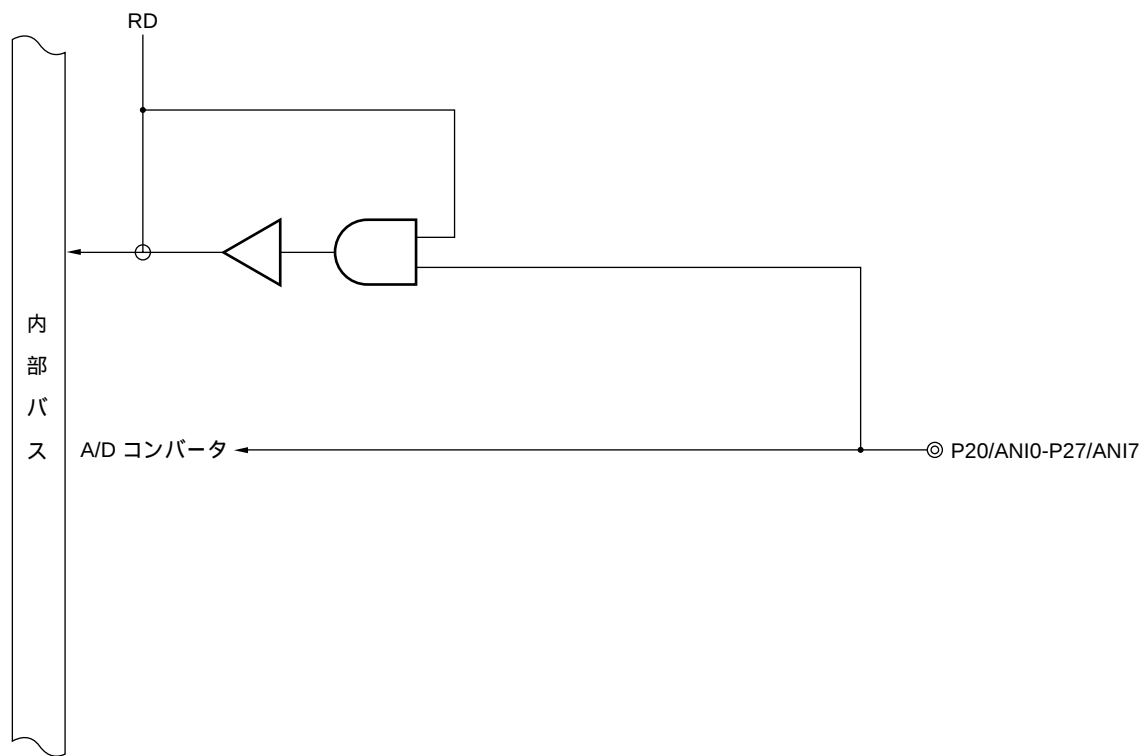
図4 - 11 P20-P27のブロック図
