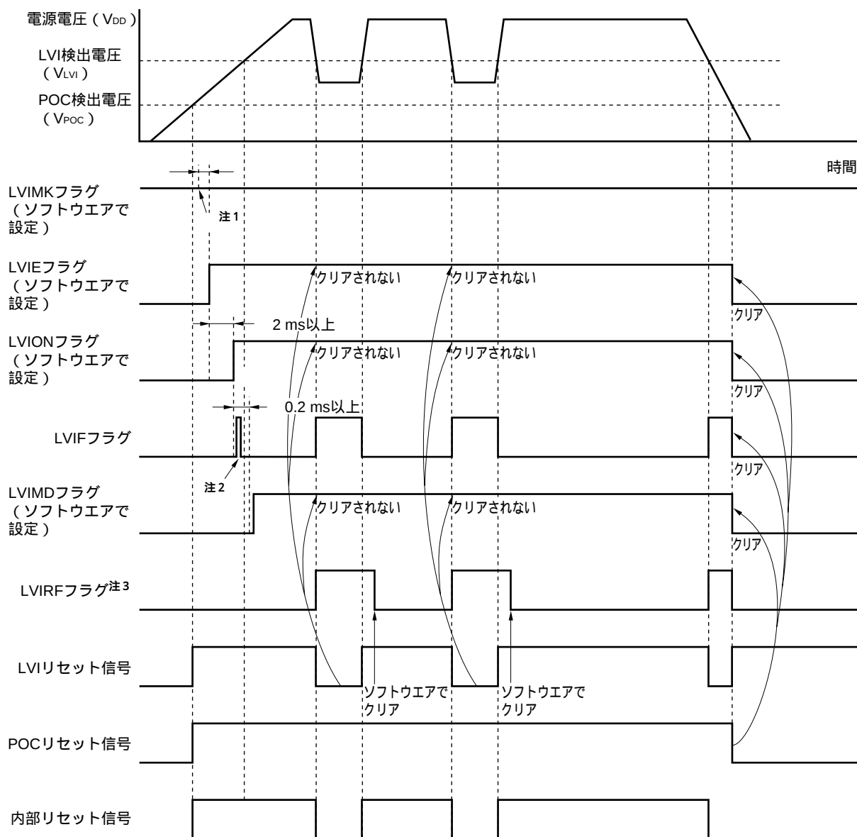
図23 - 4 低電圧検出回路の内部リセット信号発生タイミング
