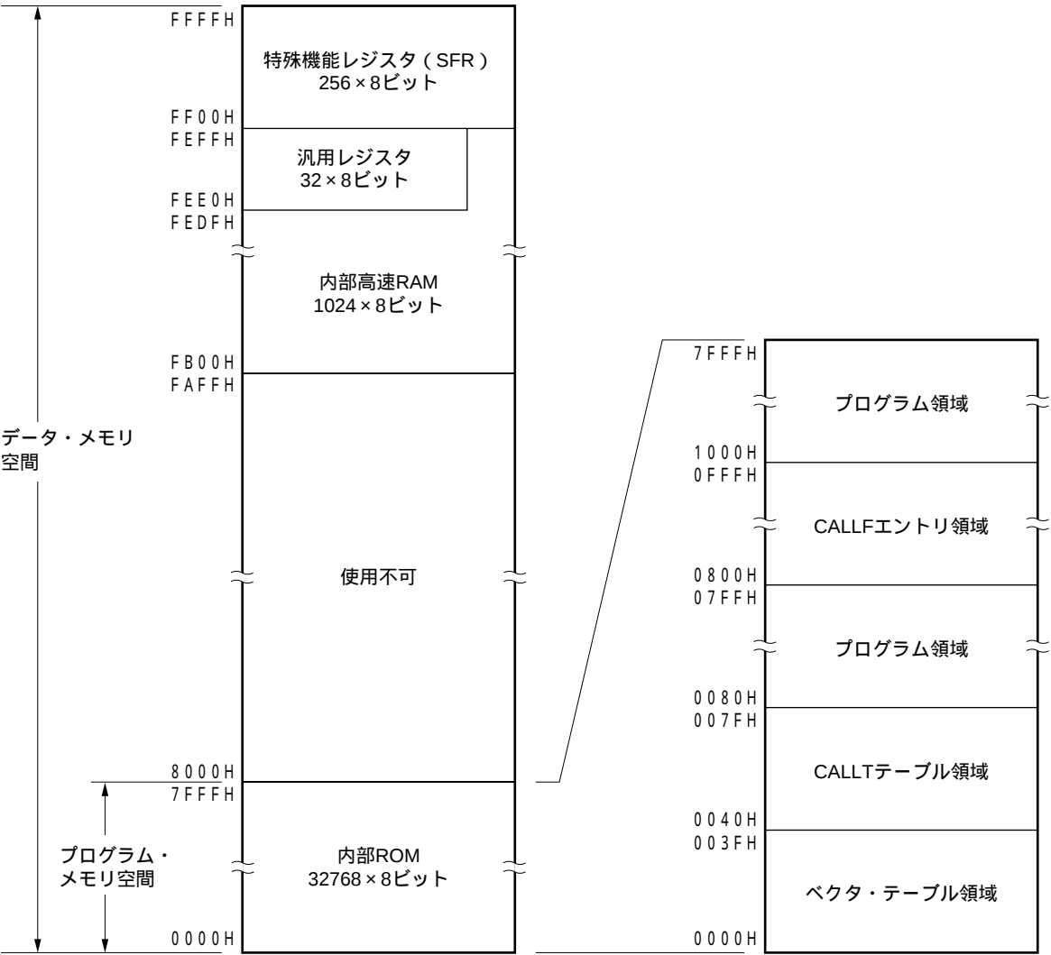
図3 - 4 メモリ・マップ (μPD780134)
