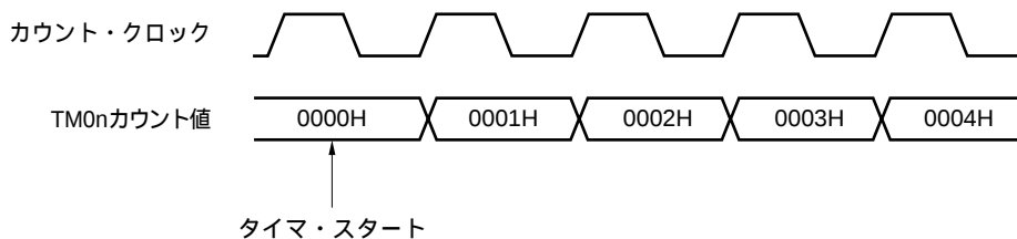
図6-40 16ビット・タイマ・カウンタ0n (TM0n) のスタート・タイミング
