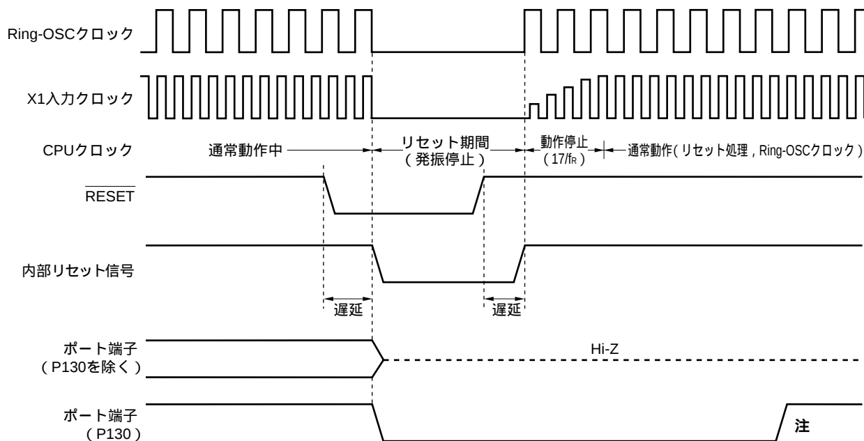
図20 - 2 RESET入力によるリセット・タイミング
