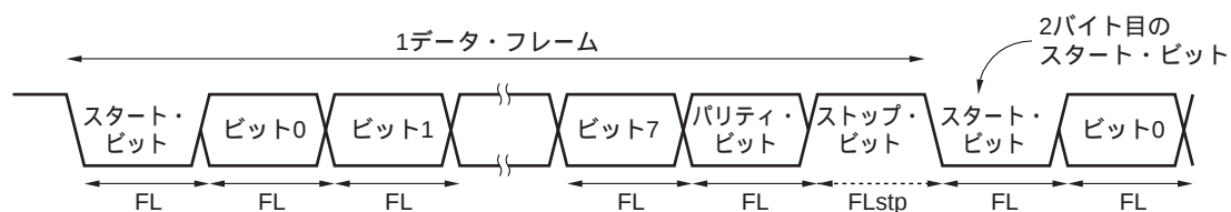
図14 - 27 連続送信時のデータ・フレーム長
