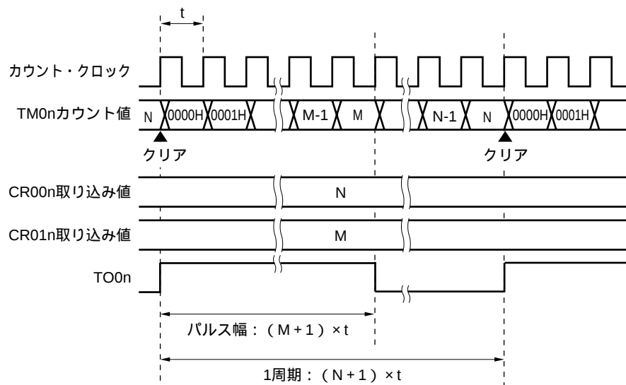
図6 - 20 PPG出力動作のタイミング
