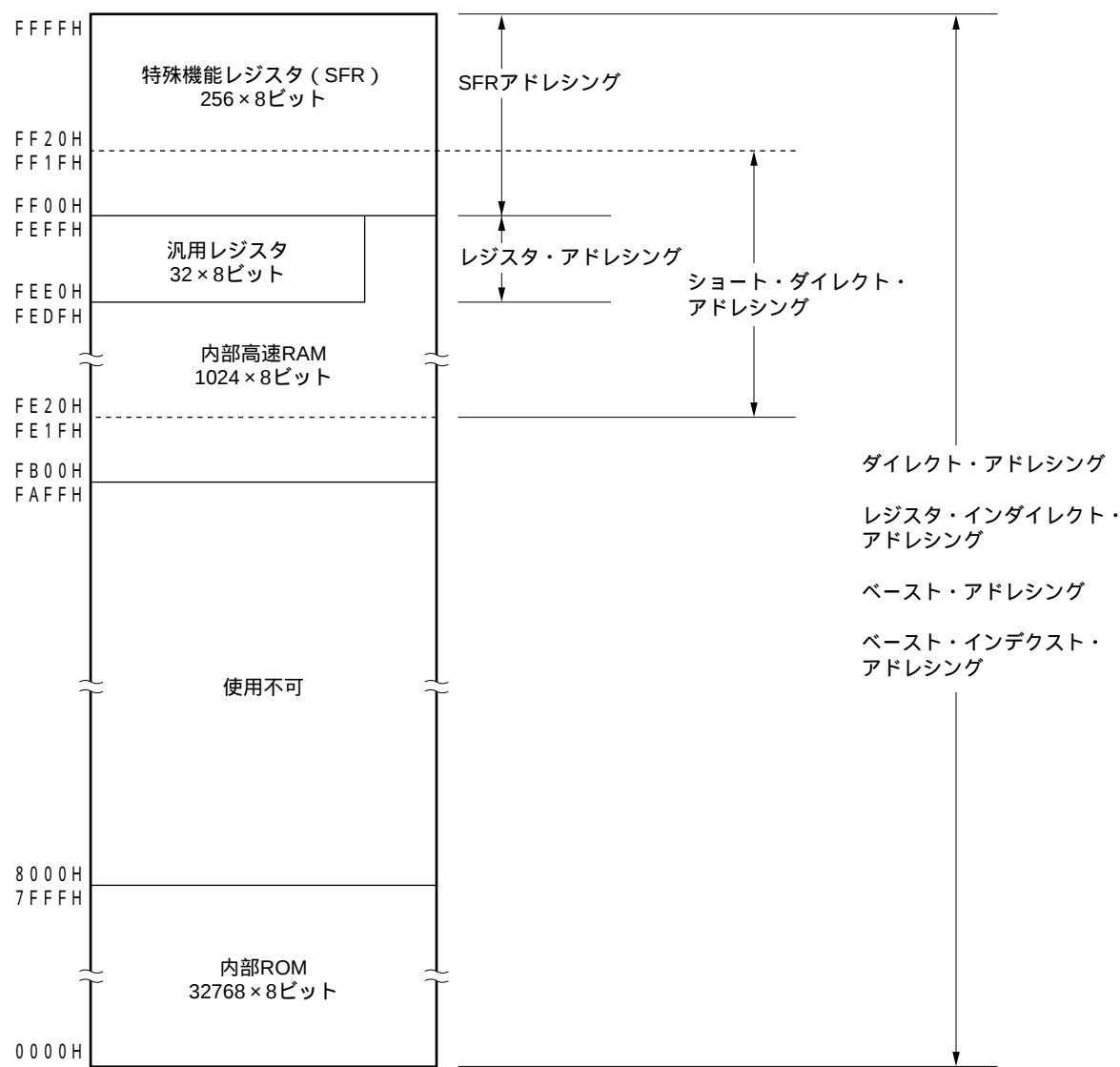
図3 - 12 データ・メモリとアドレッシングの対応 (μ PD780134)
