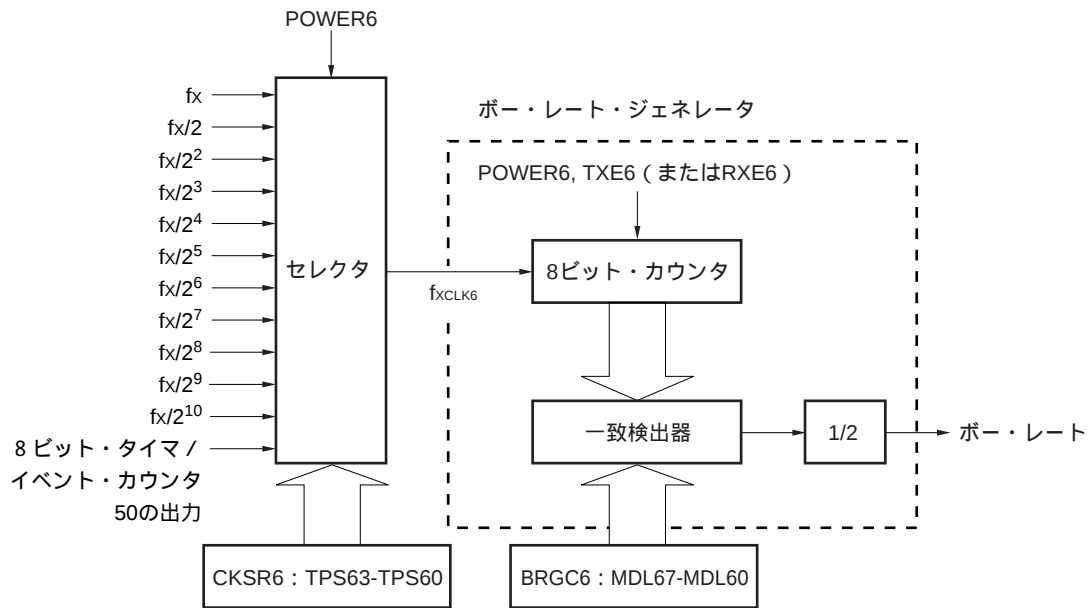
図14 - 25 ポー・レート・ジェネレータの構成
