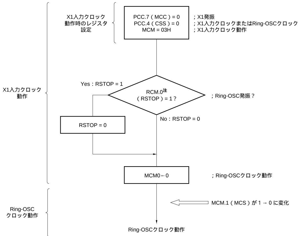
図5 - 15 X1入力クロックからRing-OSCクロックへの切り替え（フロー・チャート）
