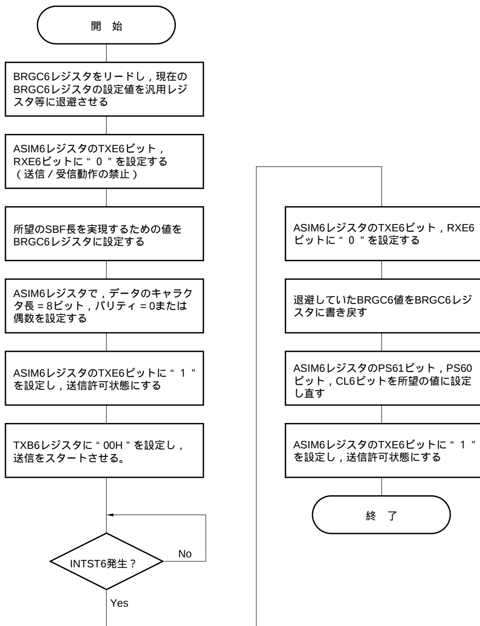
図14 - 22 SBF送信の設定手順例（フロー・チャート）
