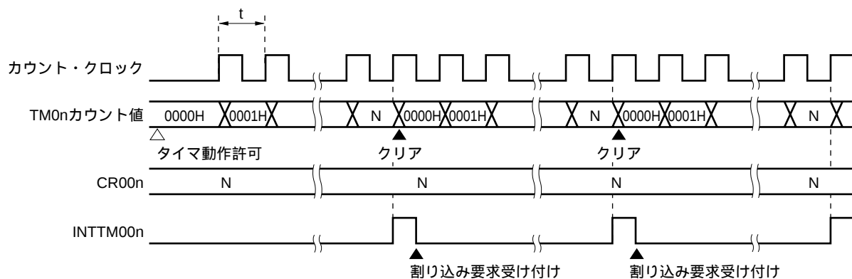
図6 - 17 インターバル・タイマ動作のタイミング
