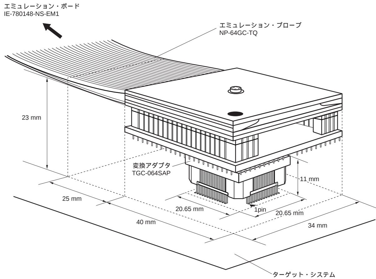
図B - 4 ターゲット・システムの接続条件 (NP-64GC-TQの場合)
