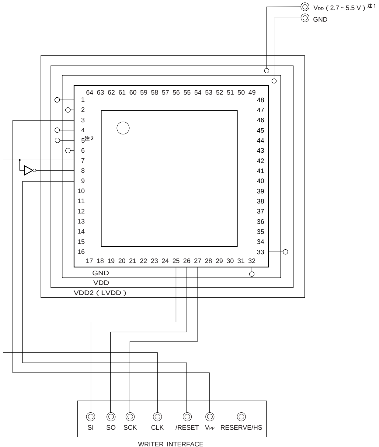
図27 - 3 3線式シリアルI/O (CSI10) 方式でのフラッシュ書き込み用アダプタ配線例
