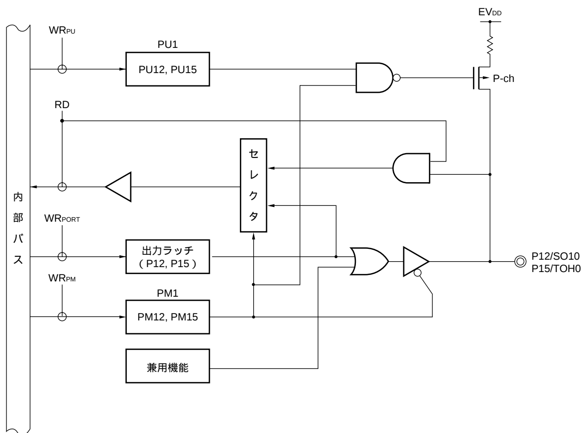
図4 - 8 P12, P15のブロック図
