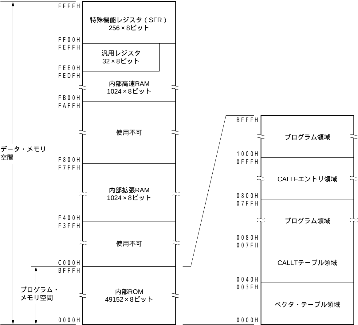
図3 - 6 メモリ・マップ (μPD780136)
