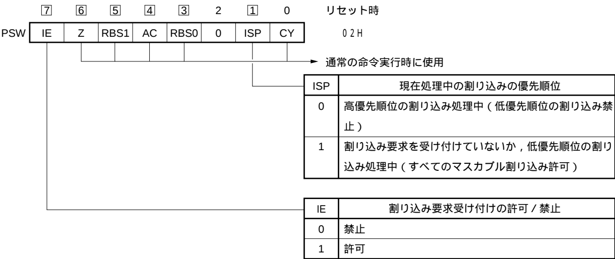
図17 - 6 プログラム・ステータス・ワードの構成
