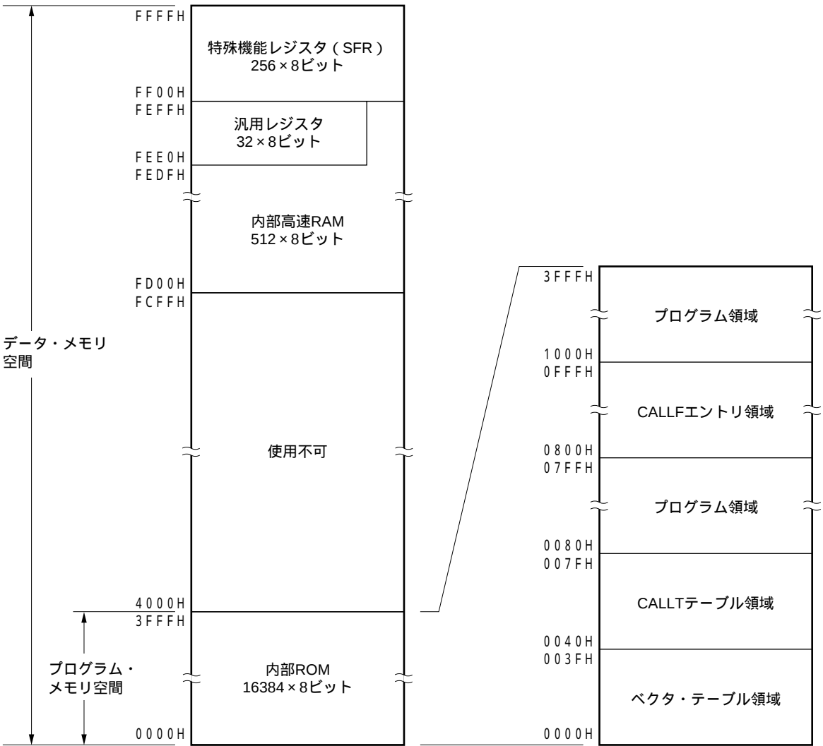
図3 - 2 メモリ・マップ (μPD780132)
