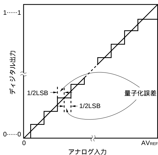
図12 - 14 量子化誤差
