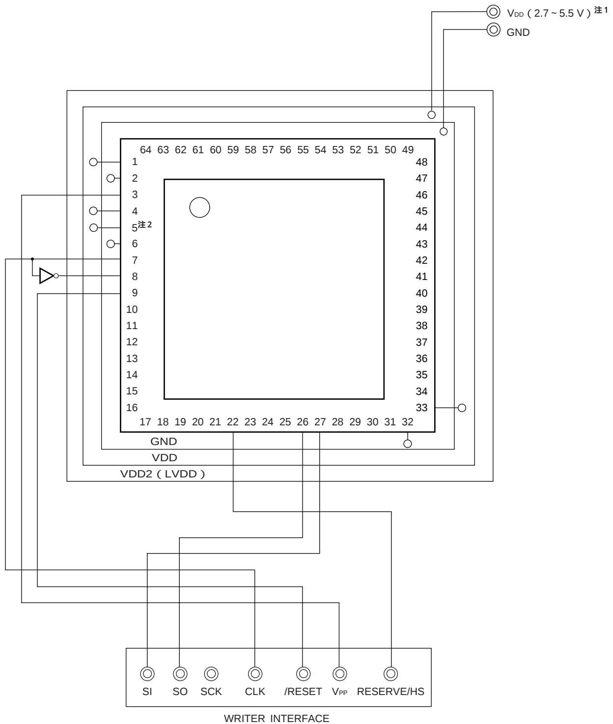
図27 - 6 UART (UART0 + HS) 方式でのフラッシュ書き込み用アダプタ配線例
