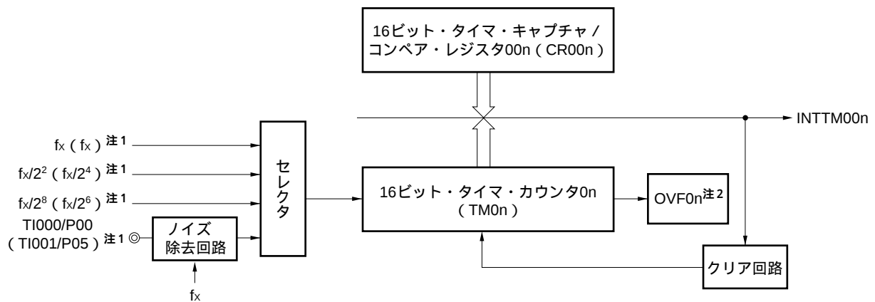
図6 - 16 インターバル・タイマの構成図
