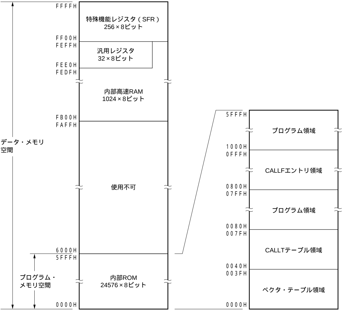
図3 - 3 メモリ・マップ (μPD780133)
