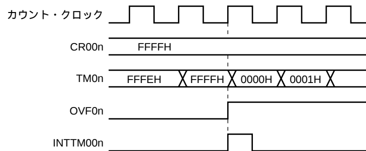
図6 - 41 OVF0nフラグの動作タイミング
