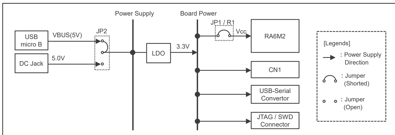
図 4 電源系統図
