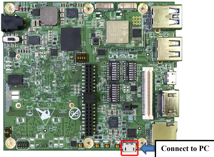
CN201:USB Type-microAB Connector
