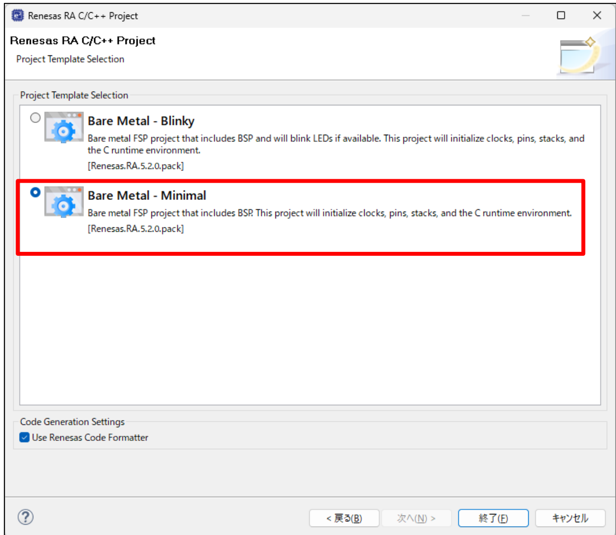
図 3-10 テンプレートタイプの設定画面
