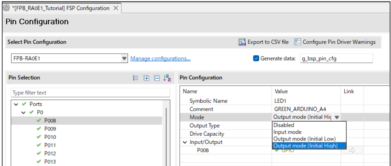
図 3-18 ピンの設定画面
