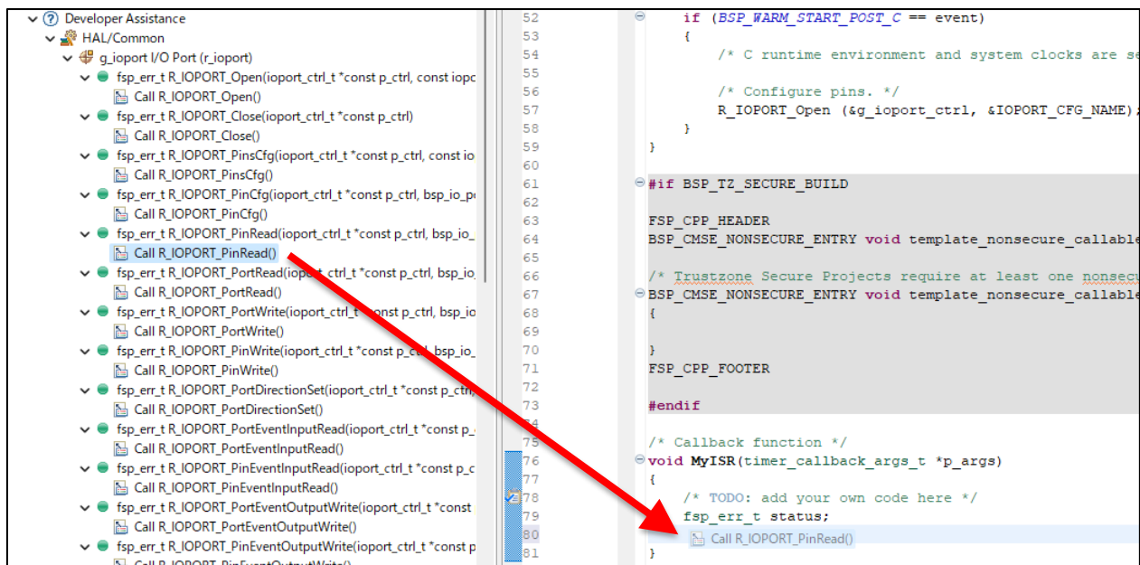
図 3-43 割り込みプログラムの実装画面
