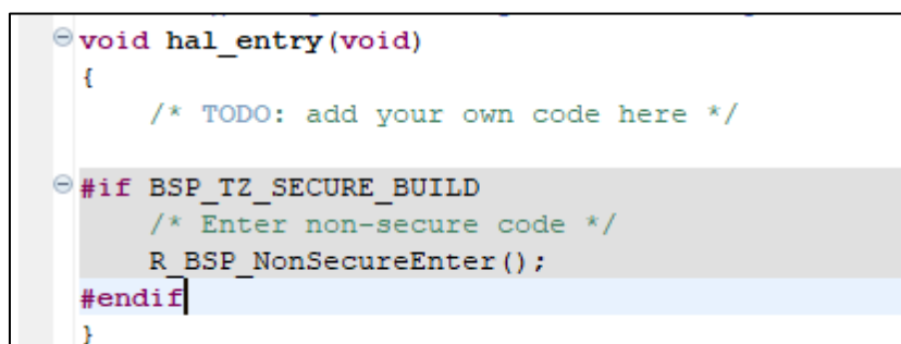
図 3-33 main プログラムの実装画面
