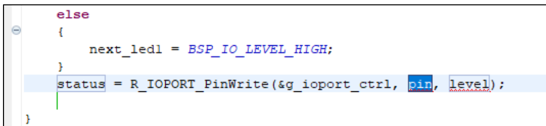
図 3-49 割り込みプログラムの実装画面
