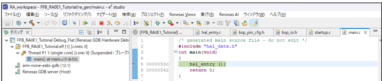
図 4-8 実行画面
