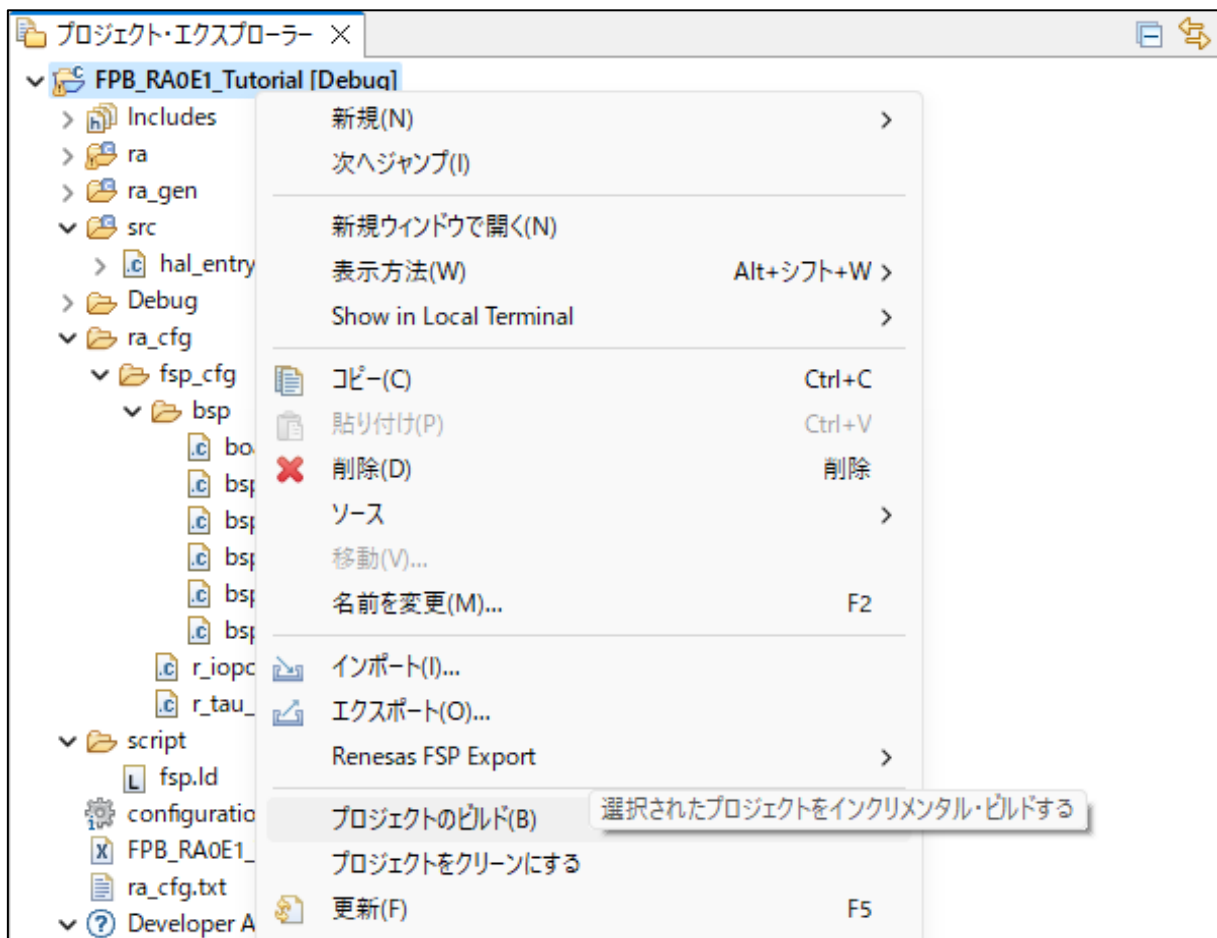
図 3-52 ビルド画面
