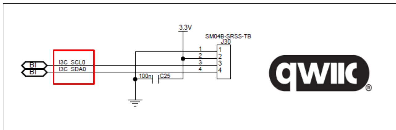
図 1 SparkFun Qwiic®コネクタの SCL および SDA のピン
