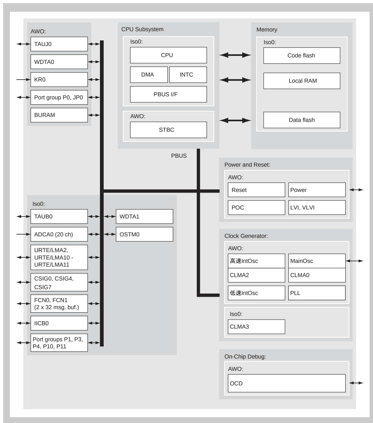
図 1-3 V850E2/FG4-L のブロック図
