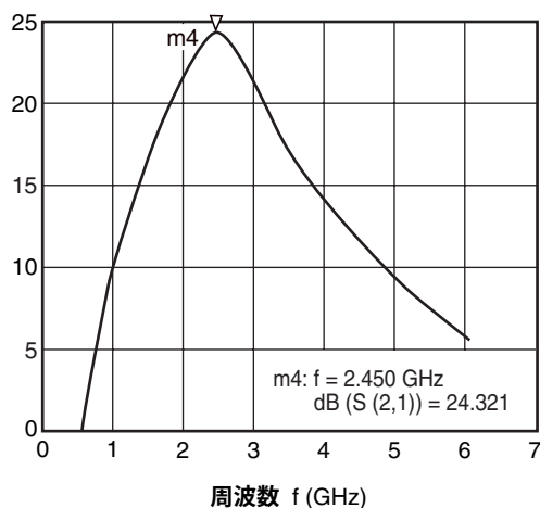
S 21 -周波数
