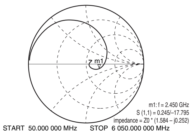
S 11 -周波数
