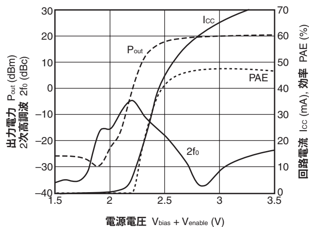
出力電力, 2次高調波, 回路電流, 効率 vs. 電源電圧
