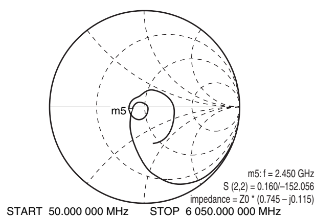
S 22 -周波数
