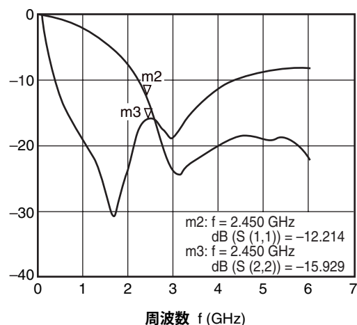
S 11 , S 22 -周波数
