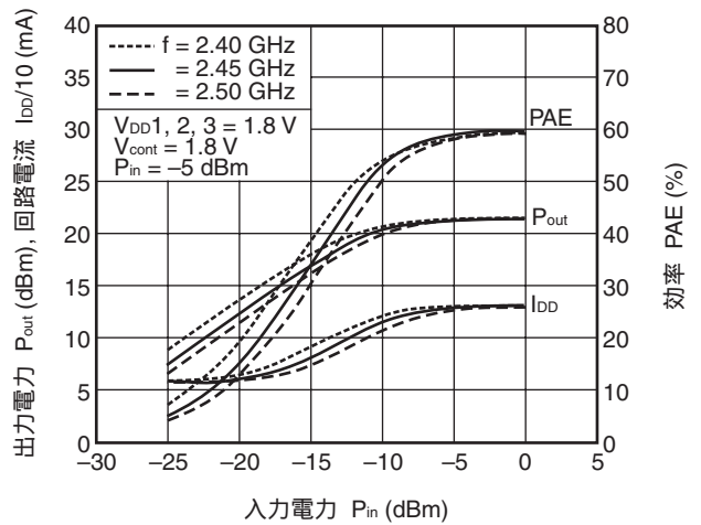
出力電力, 回路電流, 効率 vs. 入力電力
