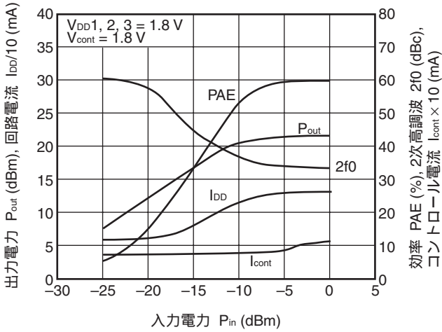
出力電力, 回路電流, 効率, 2次高調波, コントロール電流 vs. 入力電力
