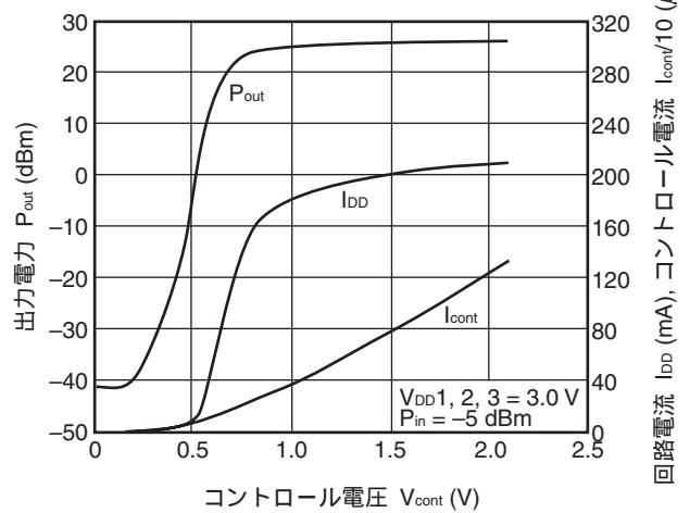
出力電力, 回路電流, コントロール電流 vs. コントロール電圧
