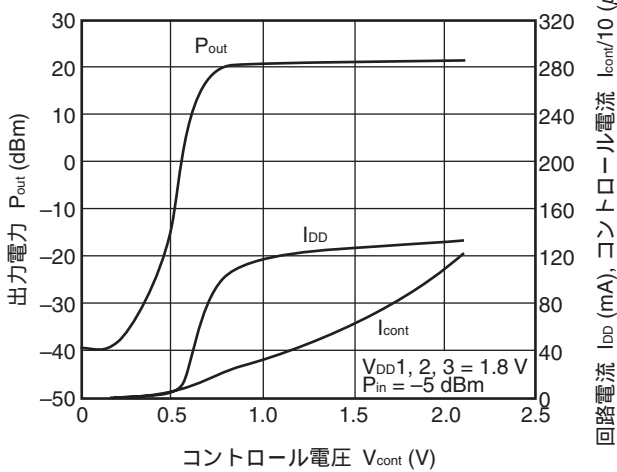
出力電力, 回路電流, コントロール電流 vs. コントロール電圧
