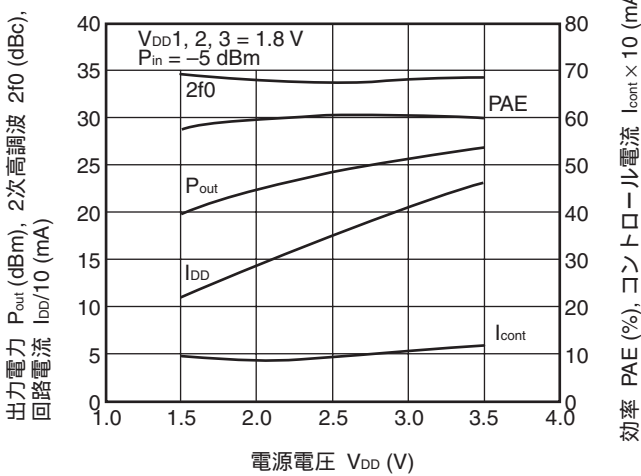
出力電力, 2次高調波, 回路電流, 効率, コントロール電流 vs. 電源電圧
