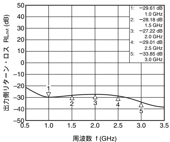
INPUT-OUTPUT1 出力側リターン・ロス vs. 周波数
