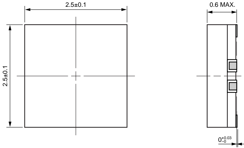
14ピン LGA (CSP 型) (単位 : mm)
