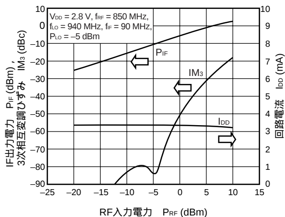
IF出力電力， IM_3 ，回路電流 vs. RF入力電力
