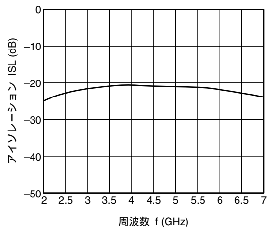
TX-RX アイソレーション vs. 周波数 (TX-ANT1 および ANT2-RX ON時)
