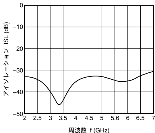
ANT2-RX アイソレーション vs. 周波数 (TX-ANT2 および ANT1-RX ON時)
