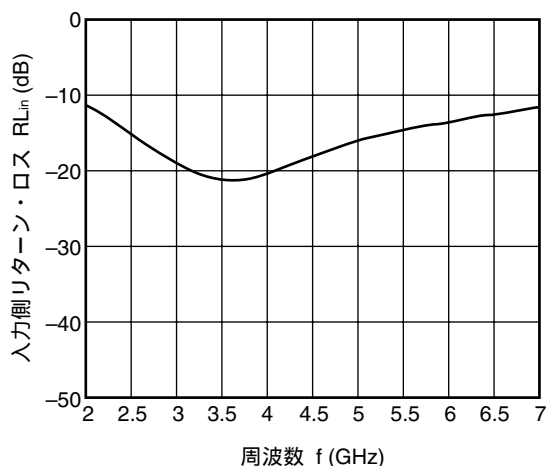
ANT2-RX 入力側リターン・ロス vs. 周波数 (TX-ANT1 および ANT2-RX ON時)
