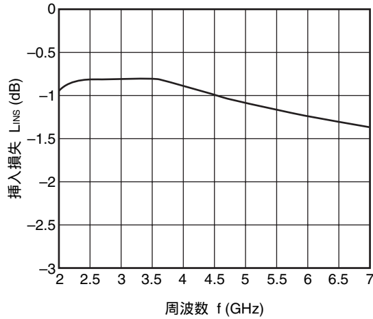
TX-ANT2 挿入損失 vs. 周波数 (TX-ANT2 および ANT1-RX ON時)
