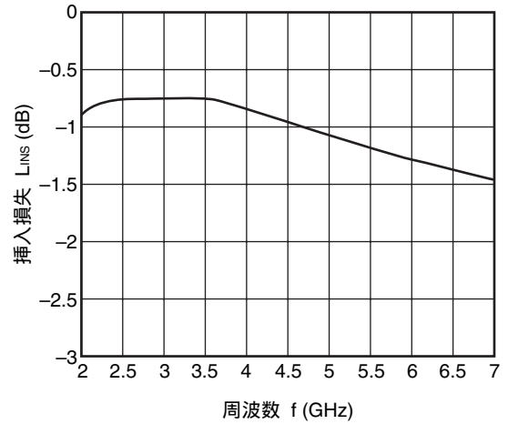
ANT2-RX 挿入損失 vs. 周波数 (TX-ANT1 および ANT2-RX ON時)
