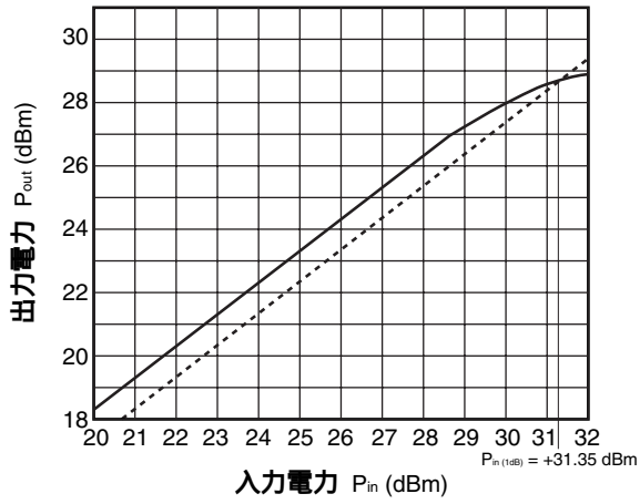
出力電力 vs. 入力電力 (f = 2.4 GHz)
