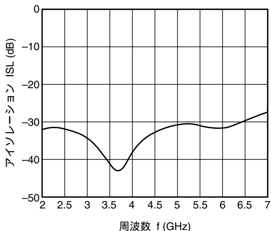
TX-ANT2 アイソレーション vs. 周波数 (TX-ANT1 および ANT2-RX ON時)
