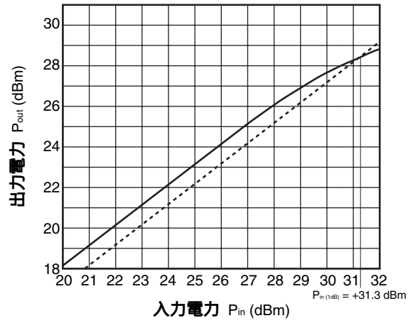
出力電力 vs. 入力電力 (f = 5.8 GHz)
