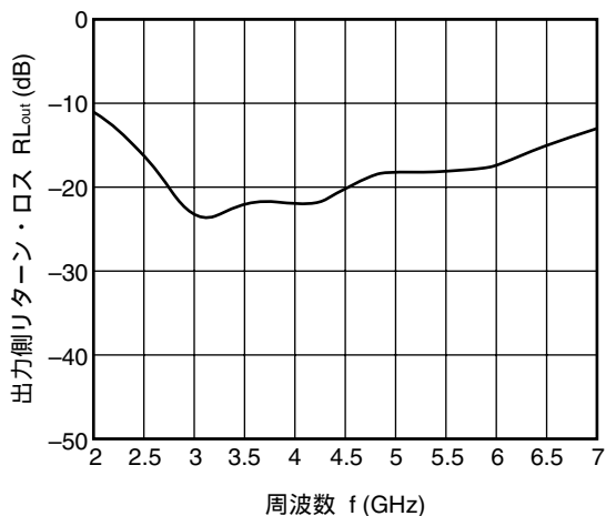
TX-ANT2 出力側リターン・ロス vs. 周波数 (TX-ANT2 および ANT1-RX ON時)
