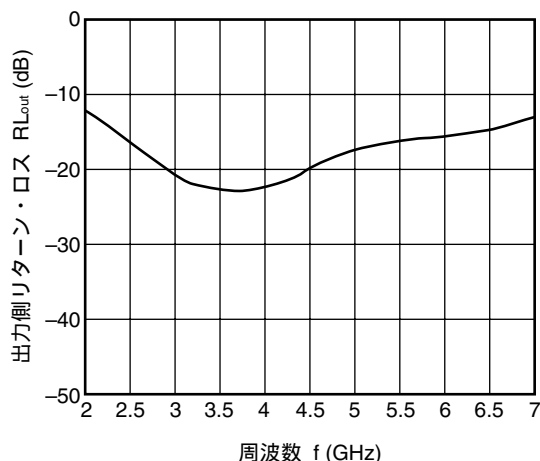
ANT1-RX 出力側リターン・ロス vs. 周波数 (TX-ANT2 および ANT1-RX ON時)
