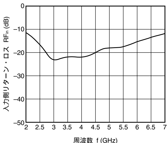
TX-ANT1 入力側リターン・ロス vs. 周波数 (TX-ANT1 および ANT2-RX ON時)
