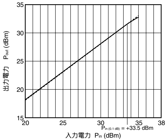
4.9 GHz 出力電力 vs. 入力電力
