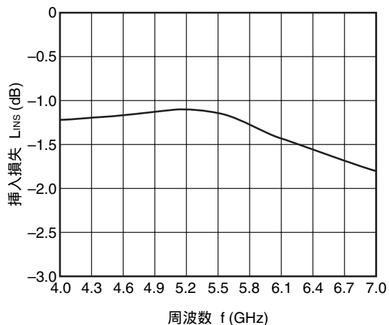
TX-ANT2 挿入損失 vs. 周波数 (TX-ANT2 ON時)
