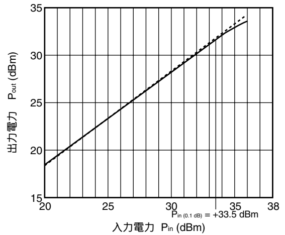
5.2 GHz 出力電力 vs. 入力電力
