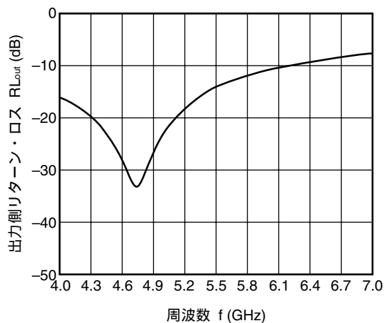
ANT1-RX 出力側リターン・ロス vs. 周波数 (ANT1-RX ON時)
