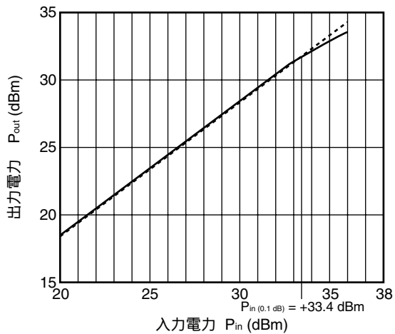
5.8 GHz 出力電力 vs. 入力電力
