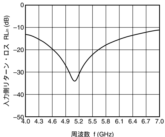
TX-ANT2 入力側リターン・ロス vs. 周波数 (TX-ANT2 ON時)
