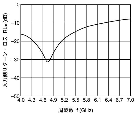
ANT1-RX 入力側リターン・ロス vs. 周波数 (ANT1-RX ON時)
