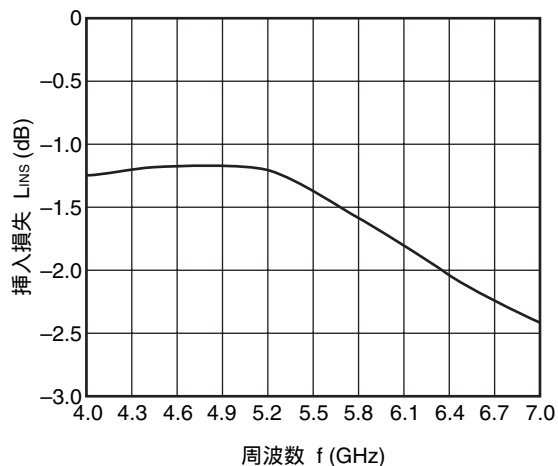
ANT2-RX 挿入損失 vs. 周波数 (ANT2-RX ON時)
