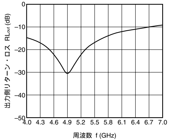
ANT2-RX 出力側リターン・ロス vs. 周波数 (ANT2-RX ON時)
