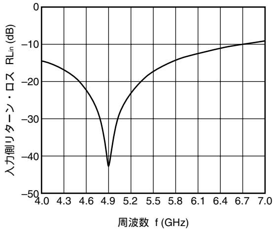
ANT2-RX 入力側リターン・ロス vs. 周波数 (ANT2-RX ON時)
