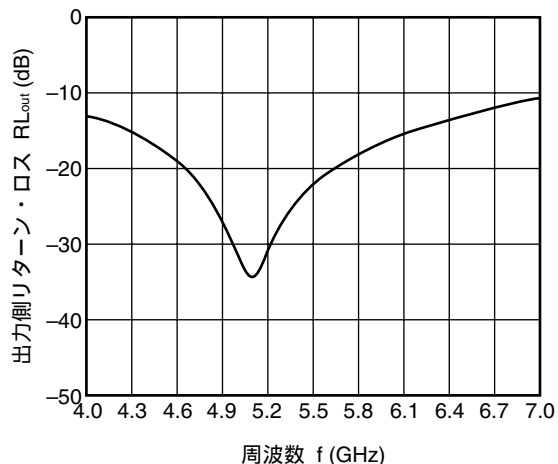
TX-ANT2 出力側リターン・ロス vs. 周波数 (TX-ANT2 ON時)
